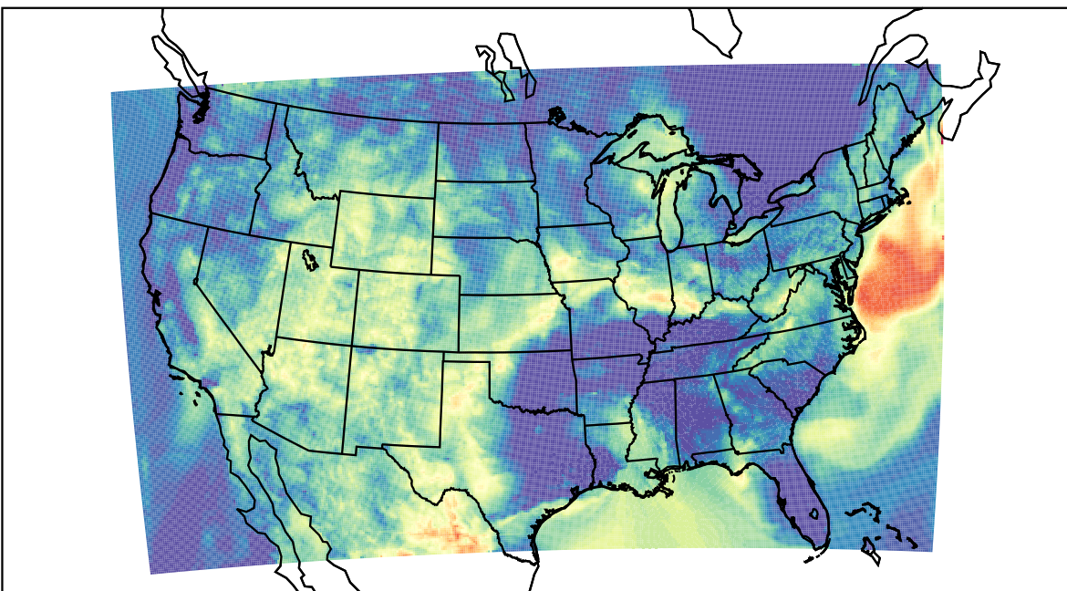
WRF (2019-07-14_11:00:00)
