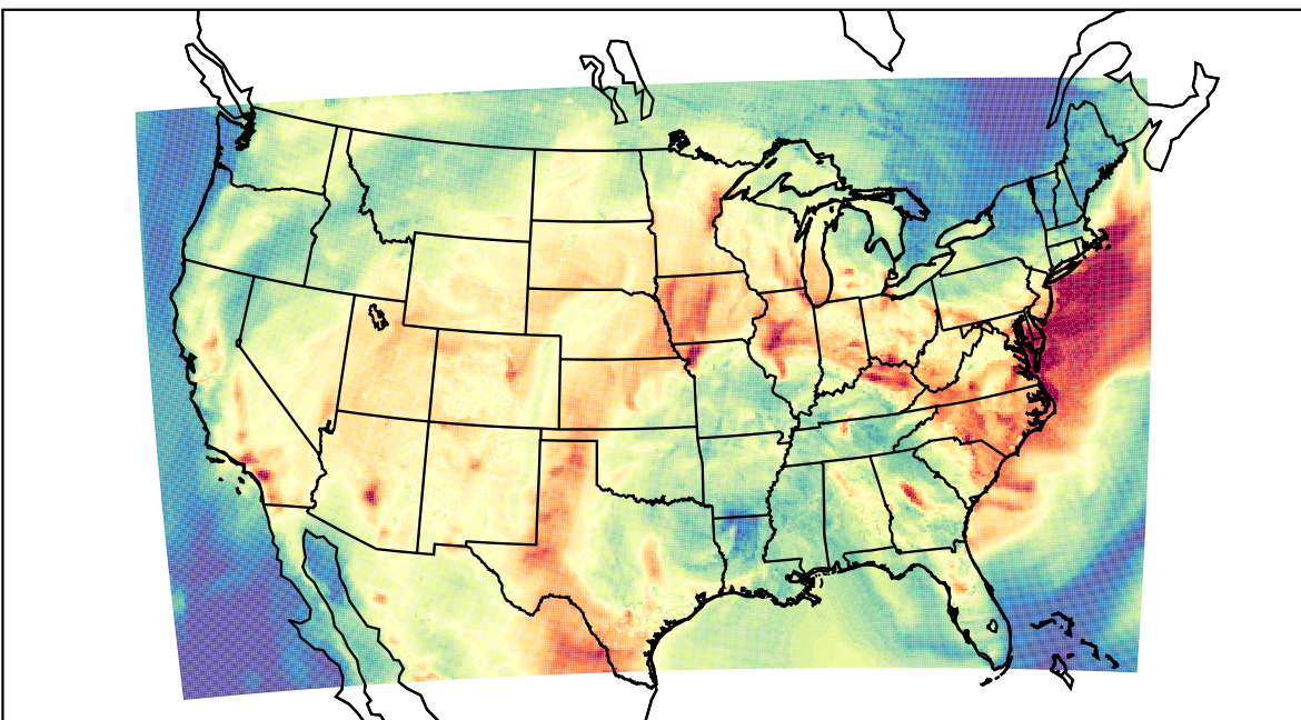
WRF (2019-07-14_22:00:00)
