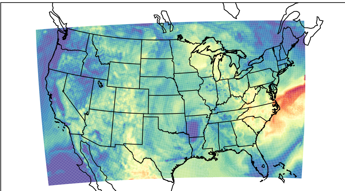
WRF (2019-07-15_14:00:00)
