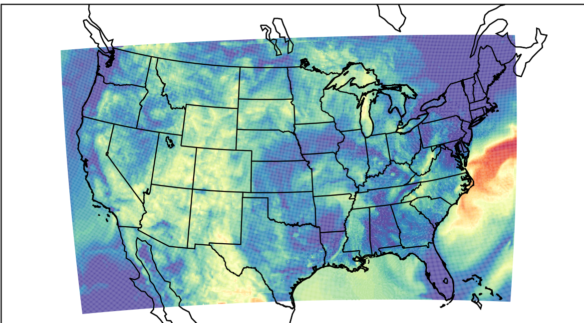
WRF (2019-07-15_11:00:00)
