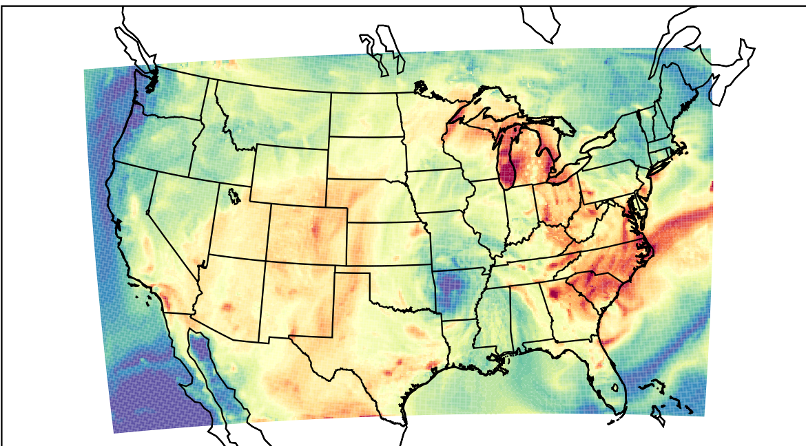
WRF (2019-07-15_19:00:00)
