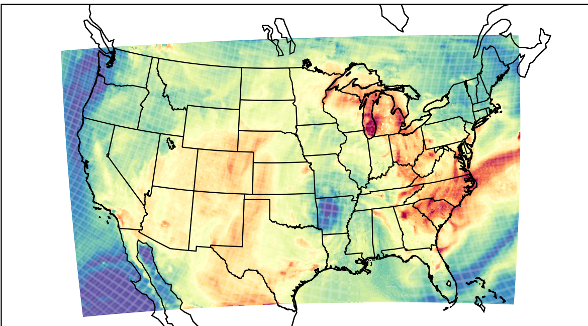
WRF (2019-07-15_18:00:00)
