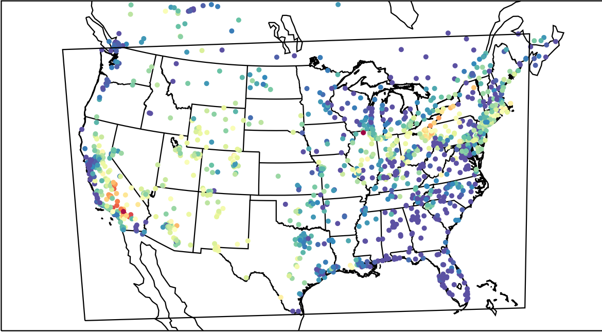
AirNOW (2019-07-14_03:00:00)
