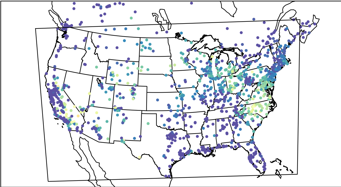
AirNOW (2019-07-15_13:00:00)
