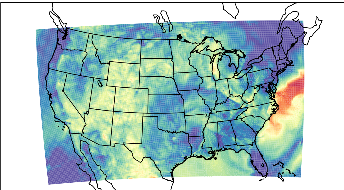
WRF (2019-07-15_08:00:00)
