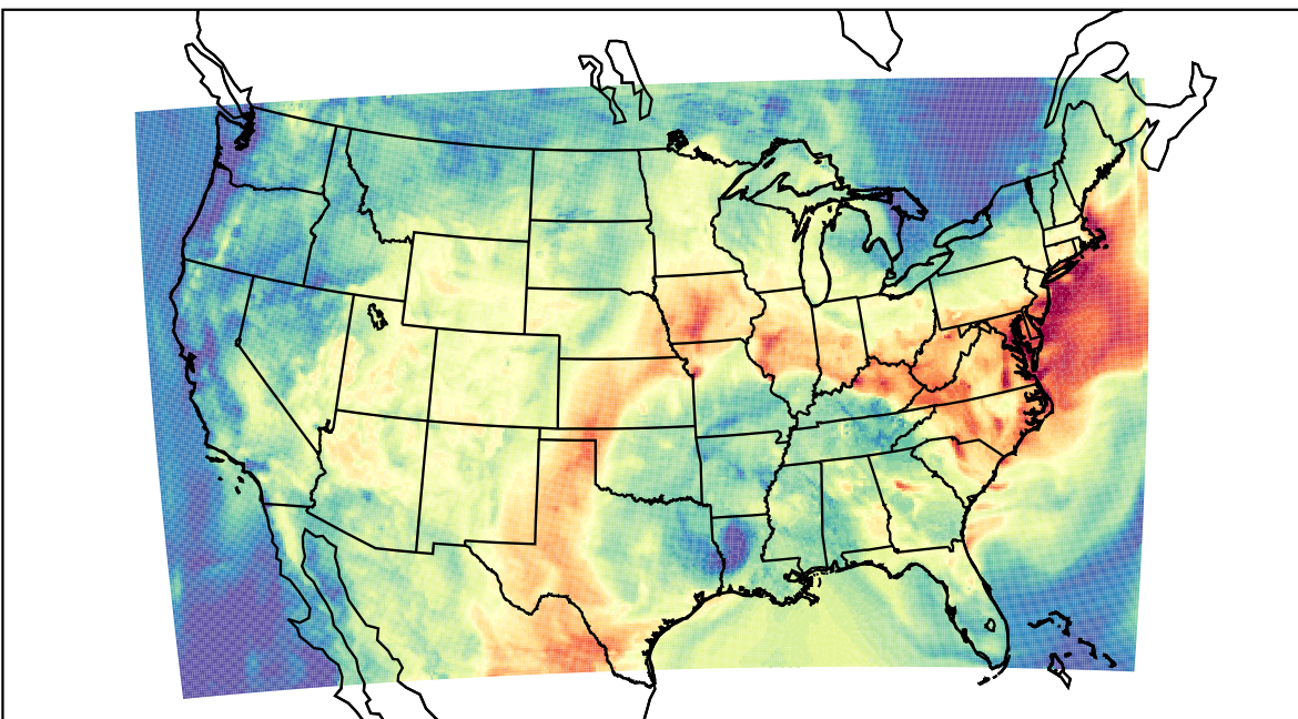
WRF (2019-07-14_16:00:00)
