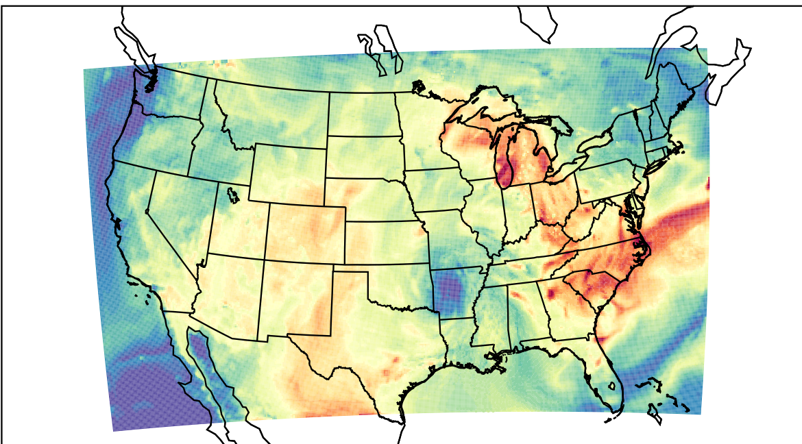
WRF (2019-07-15_17:00:00)
