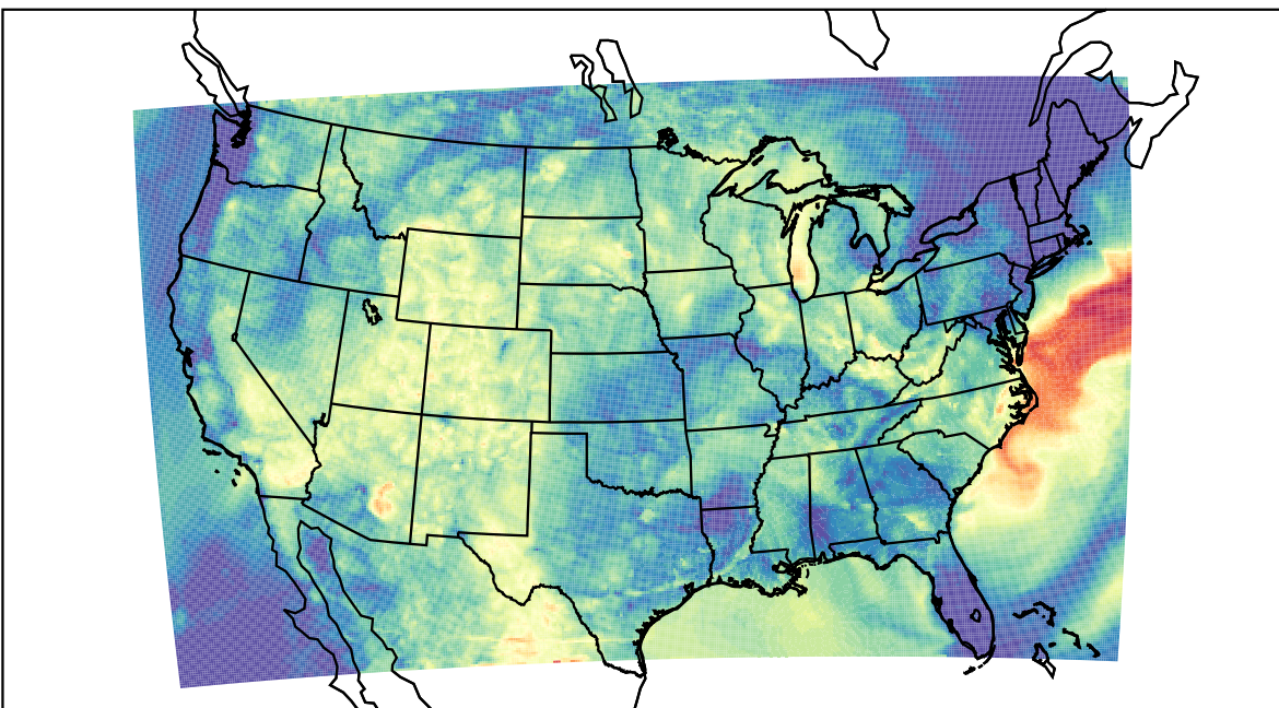
WRF (2019-07-15_06:00:00)
