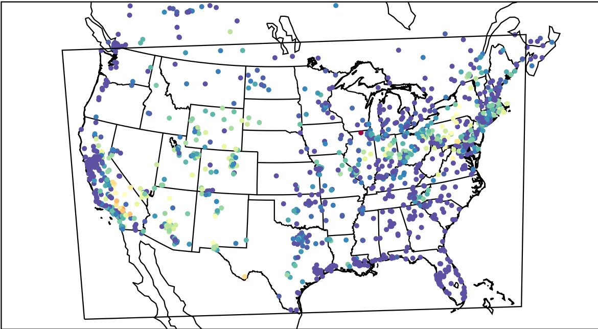
AirNOW (2019-07-14_08:00:00)
