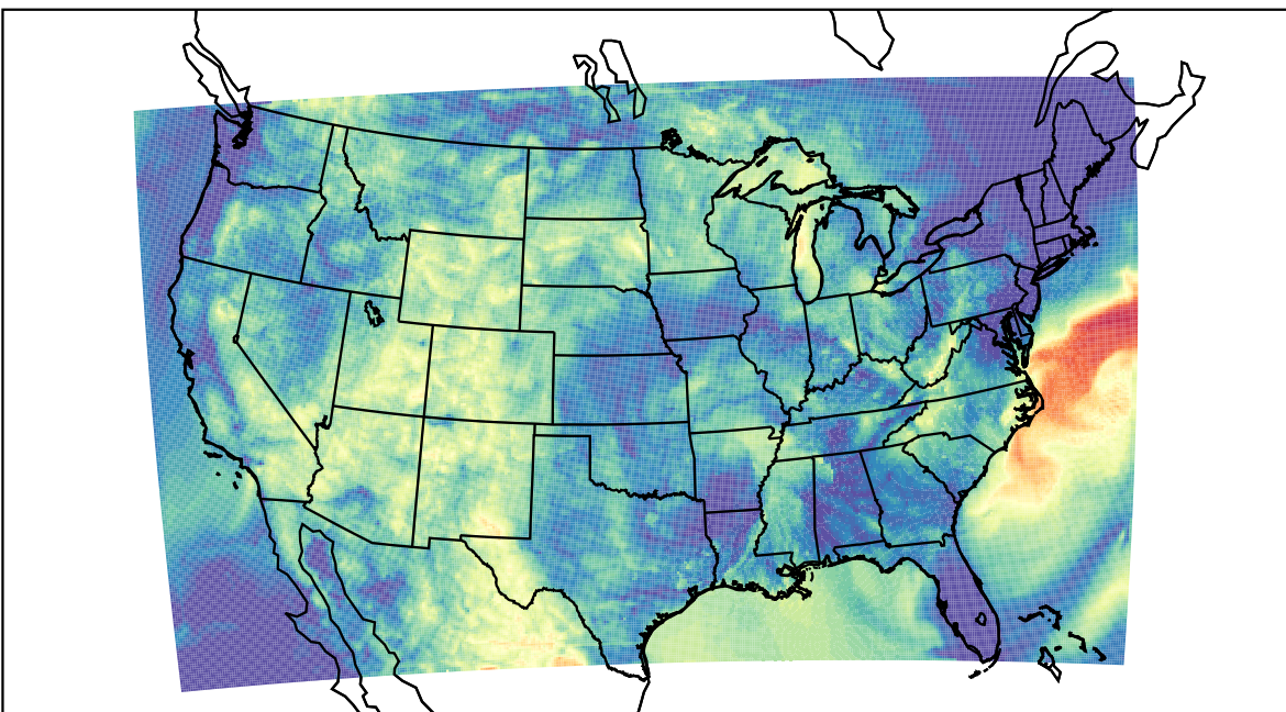
WRF (2019-07-15_10:00:00)
