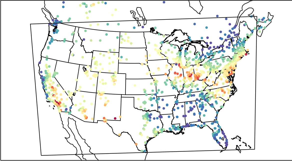
AirNOW (2019-07-14_19:00:00)
