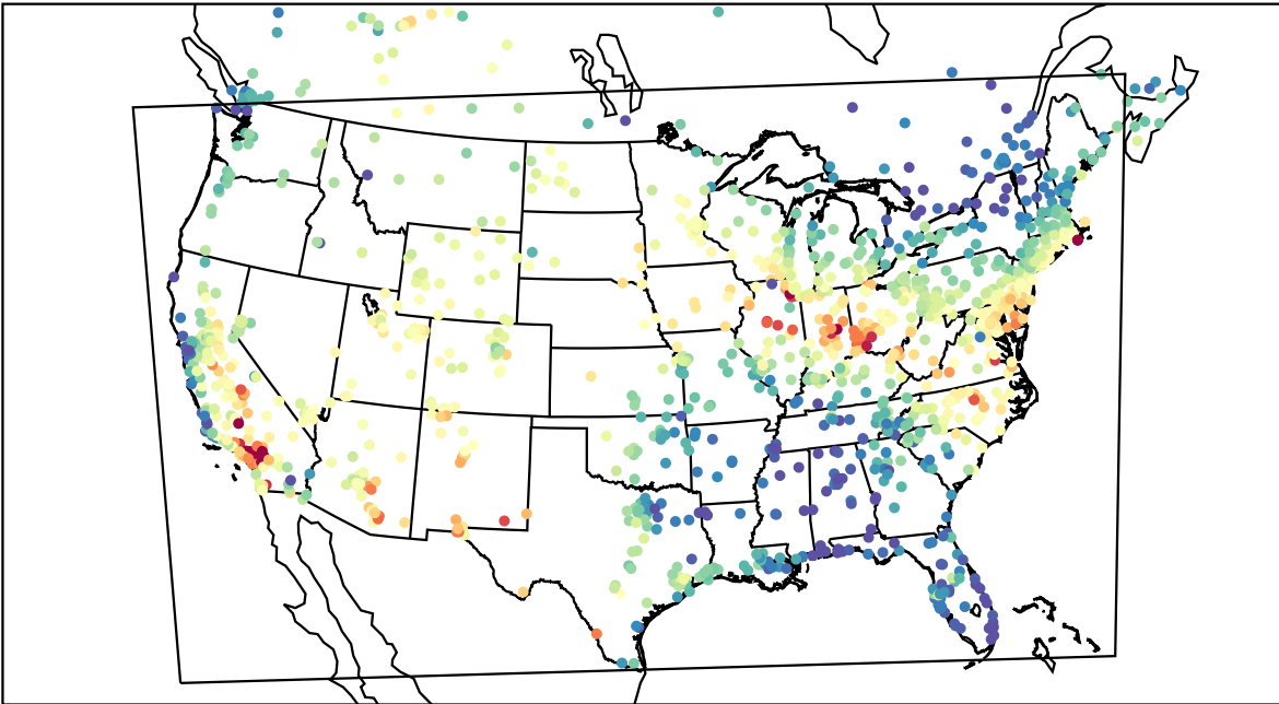
AirNOW (2019-07-14_21:00:00)
