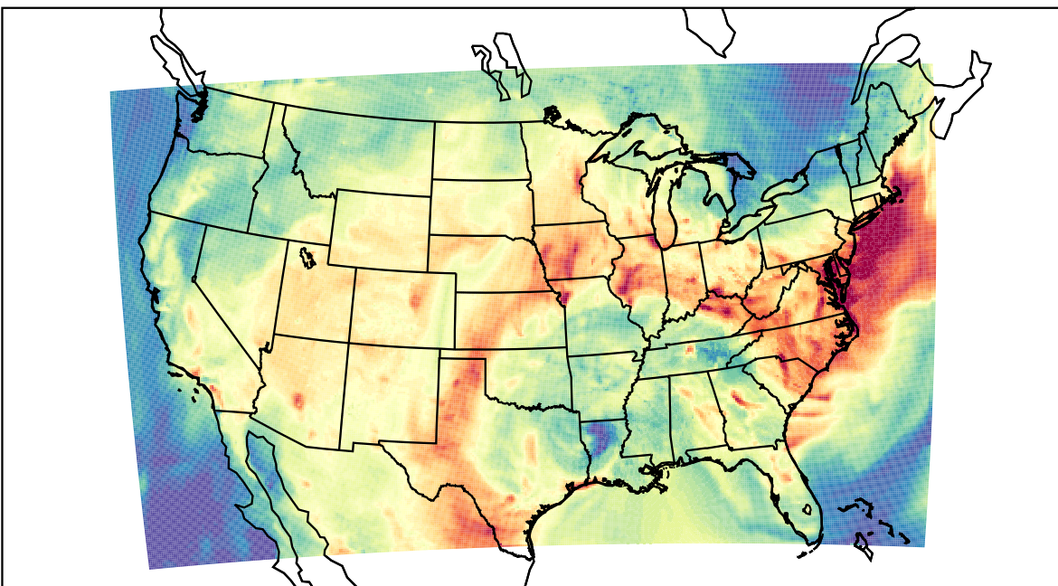
WRF (2019-07-14_19:00:00)
