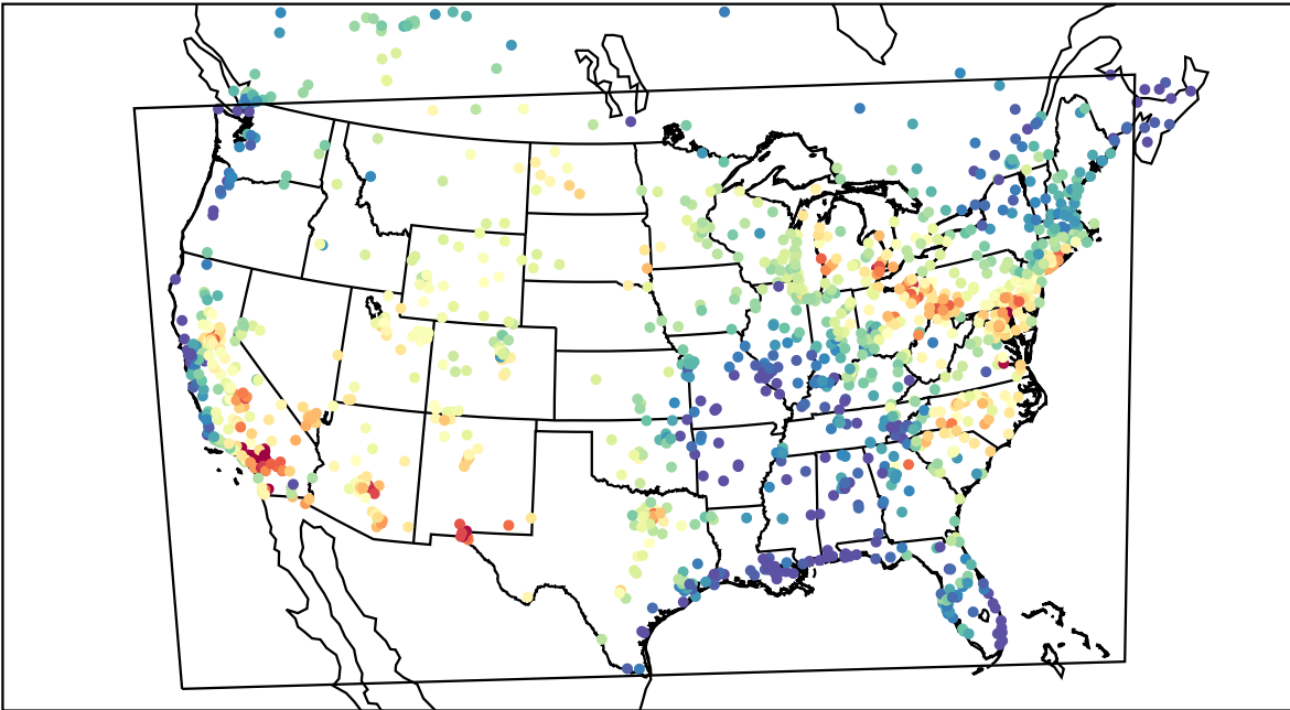
AirNOW (2019-07-15_22:00:00)
