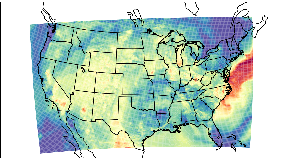
WRF (2019-07-15_03:00:00)
