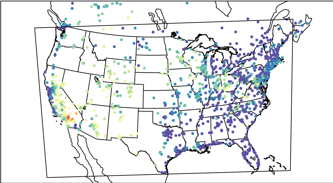
AirNOW (2019-07-15_03:00:00)
