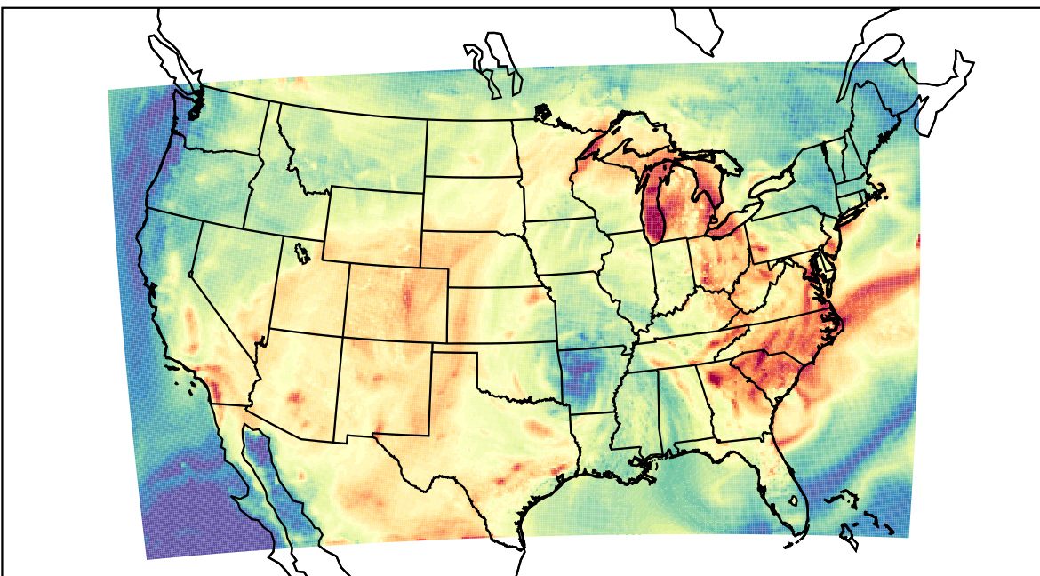
WRF (2019-07-15_20:00:00)
