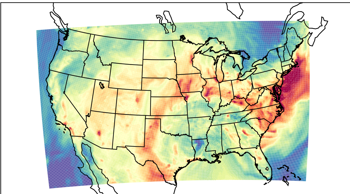
WRF (2019-07-14_20:00:00)
