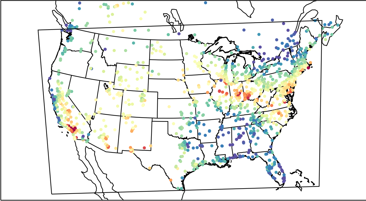
AirNOW (2019-07-14_20:00:00)
