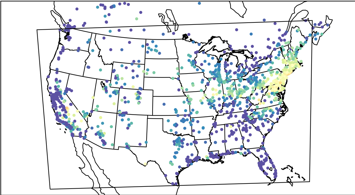
AirNOW (2019-07-14_13:00:00)
