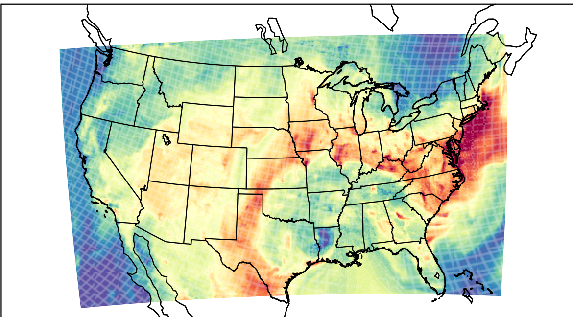
WRF (2019-07-14_18:00:00)
