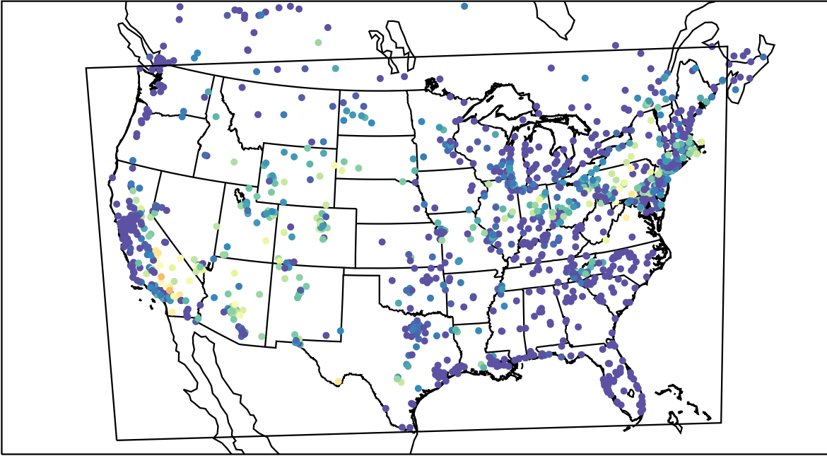
AirNOW (2019-07-14_09:00:00)
