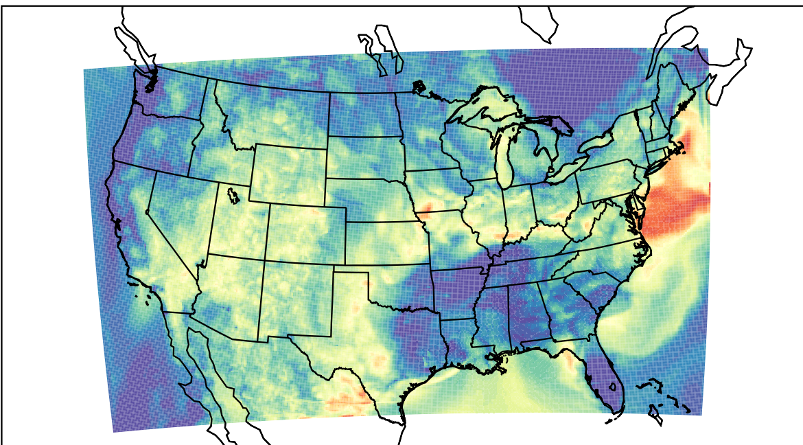
WRF (2019-07-14_06:00:00)
