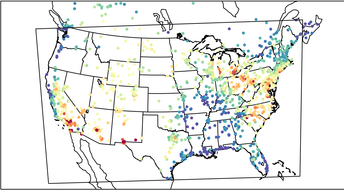
AirNOW (2019-07-15_20:00:00)
