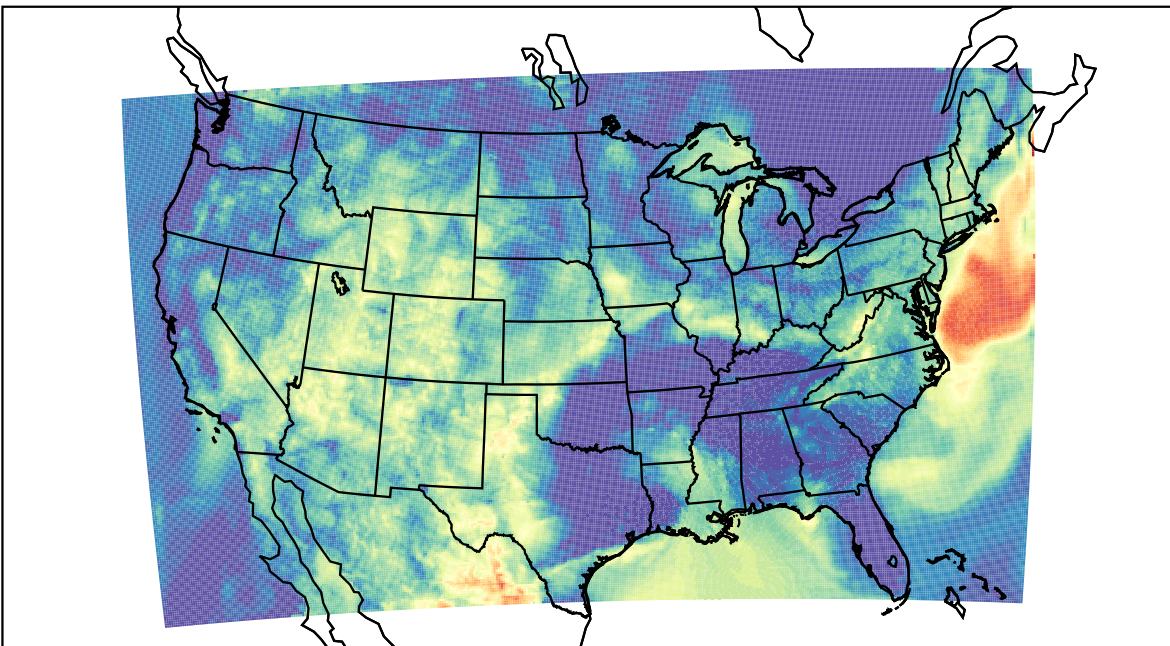
WRF (2019-07-14_12:00:00)
