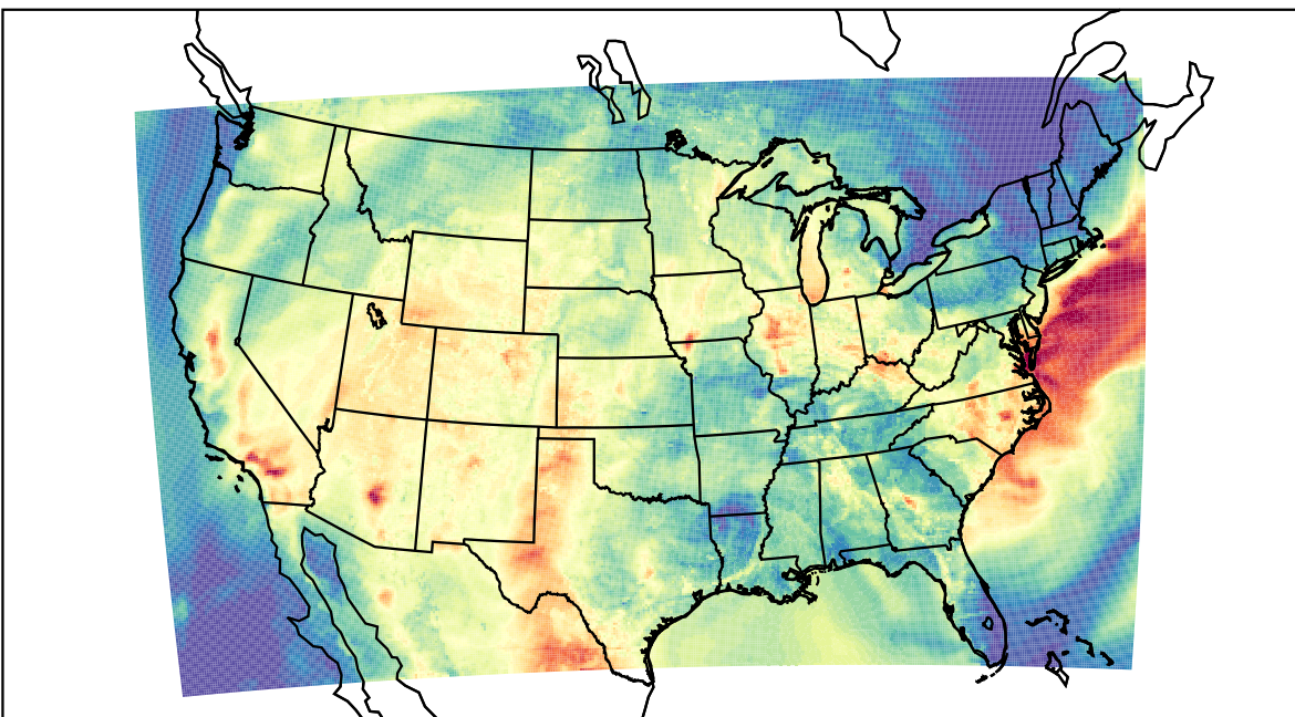
WRF (2019-07-15_01:00:00)
