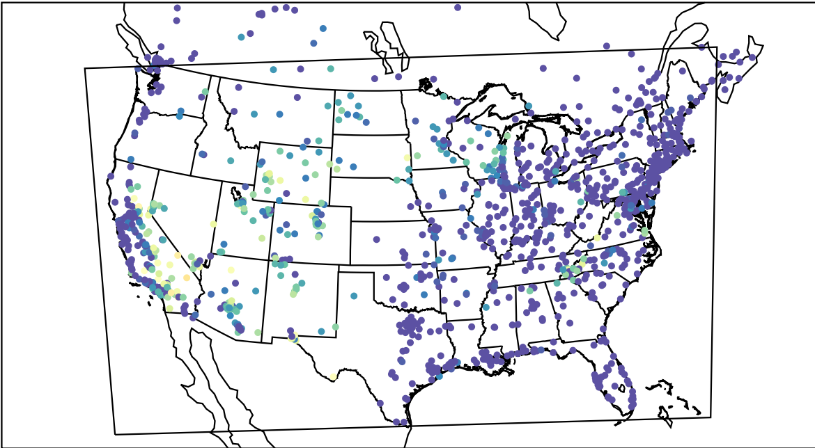
AirNOW (2019-07-15_10:00:00)
