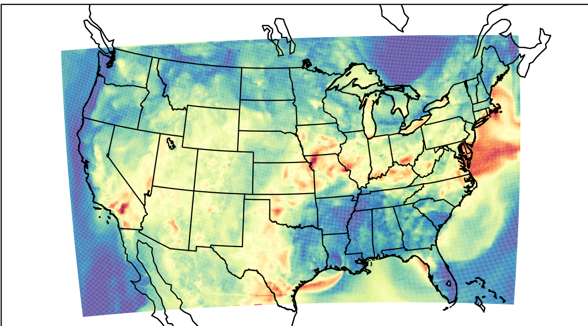
WRF (2019-07-14_02:00:00)
