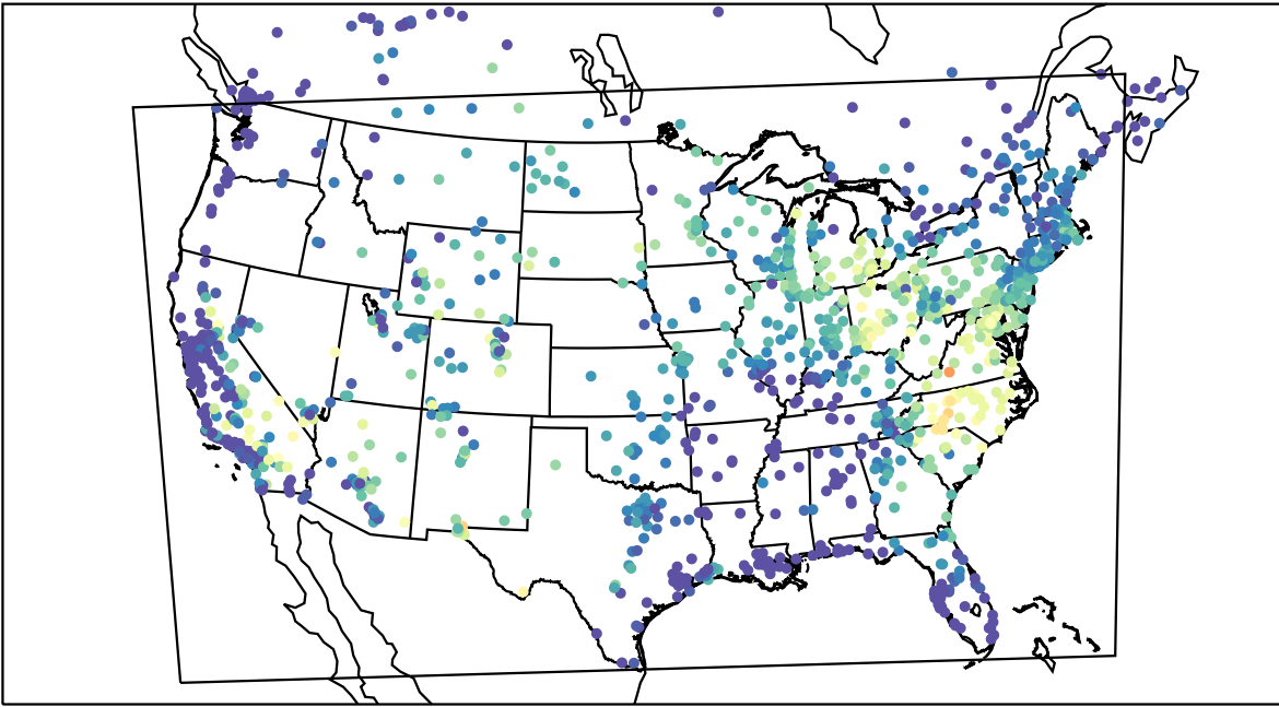
AirNOW (2019-07-15_14:00:00)
