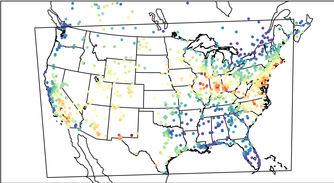
AirNOW (2019-07-14_18:00:00)
