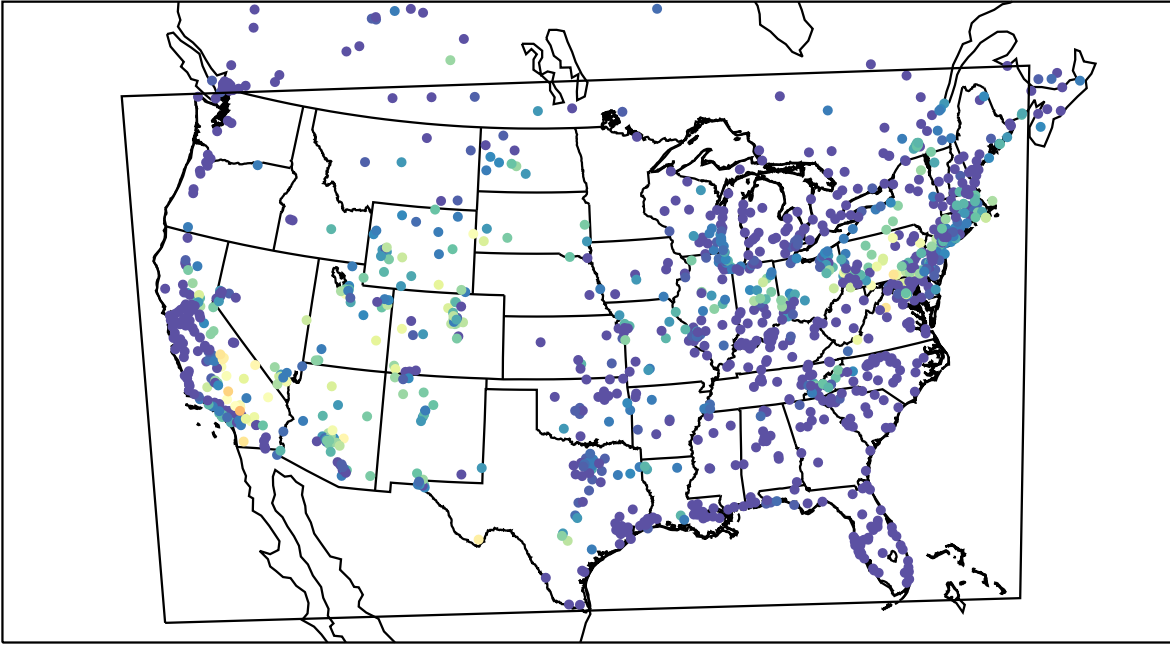
AirNOW (2019-07-14_10:00:00)
