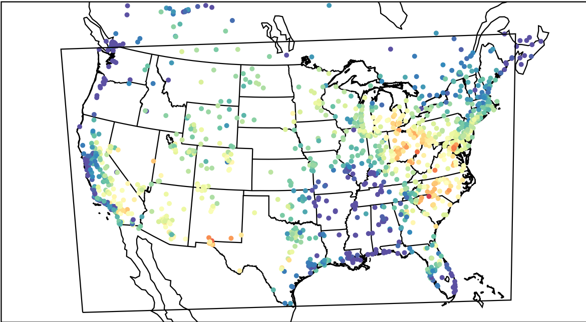
AirNOW (2019-07-15_16:00:00)
