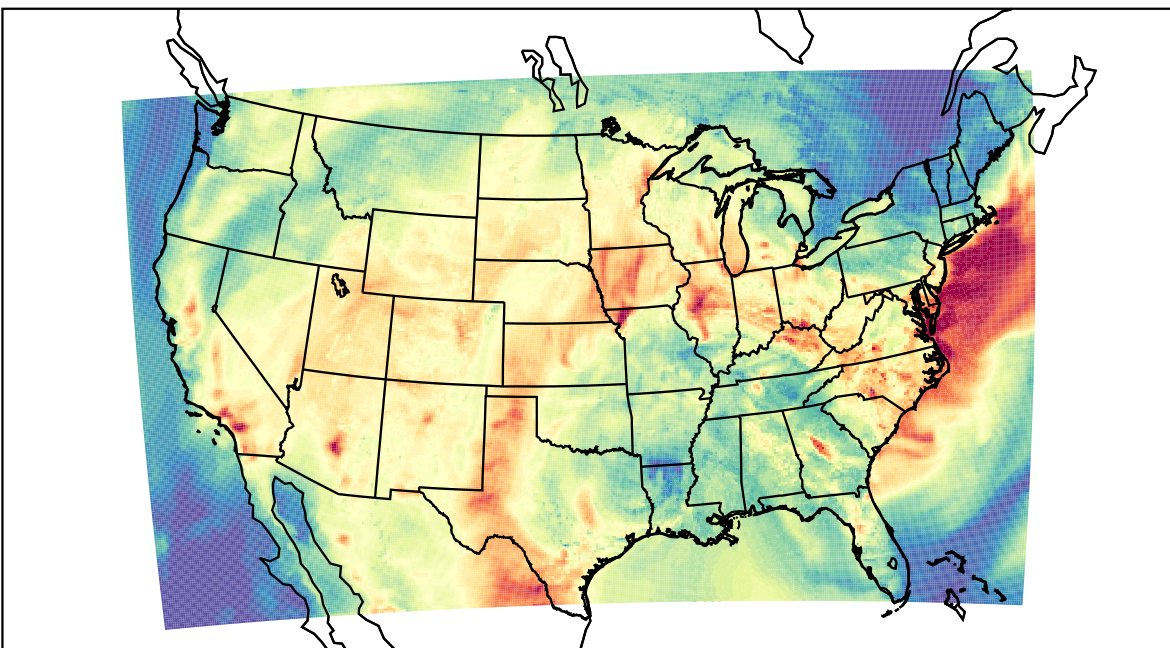
WRF (2019-07-14_23:00:00)
