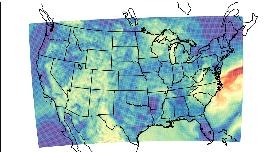
WRF (2019-07-15_13:00:00)
