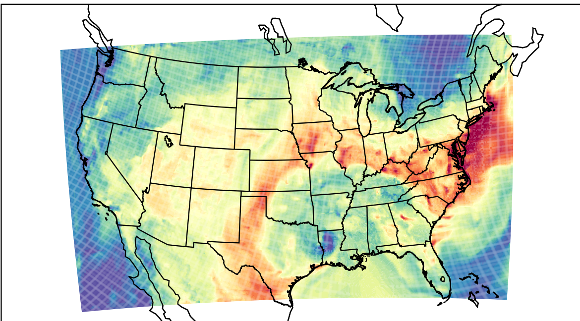
WRF (2019-07-14_17:00:00)
