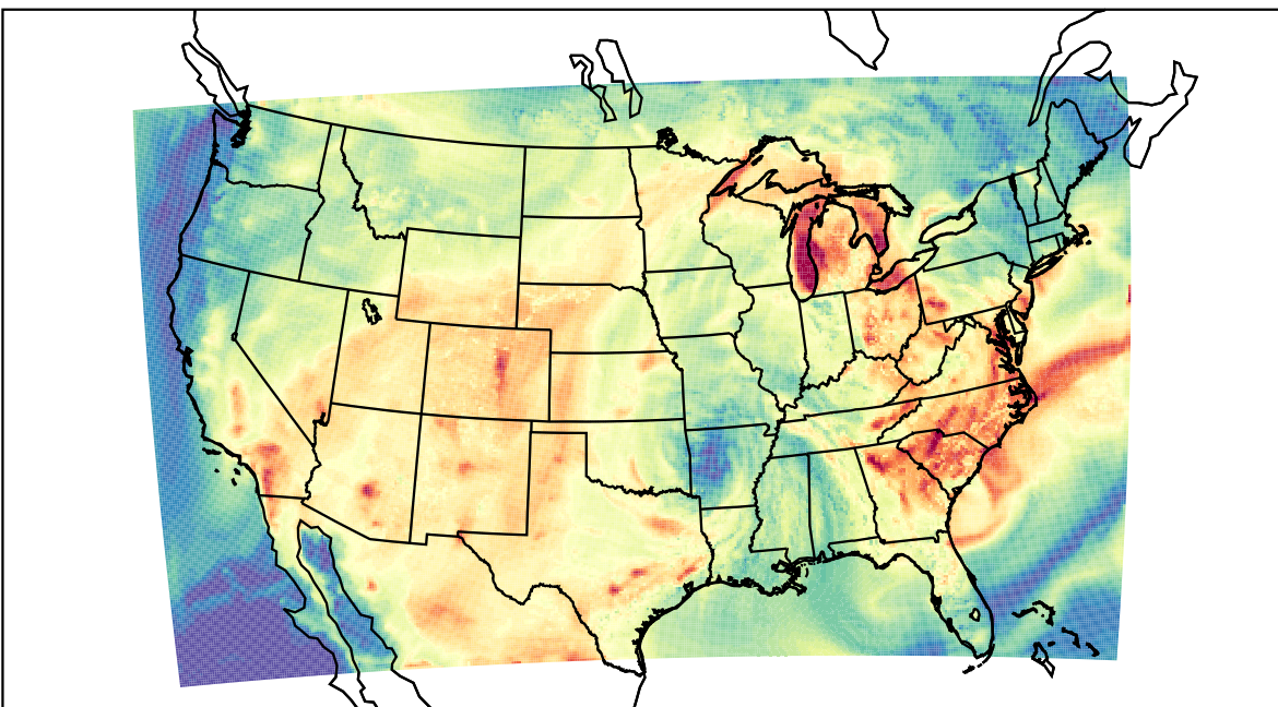
WRF (2019-07-15_22:00:00)
