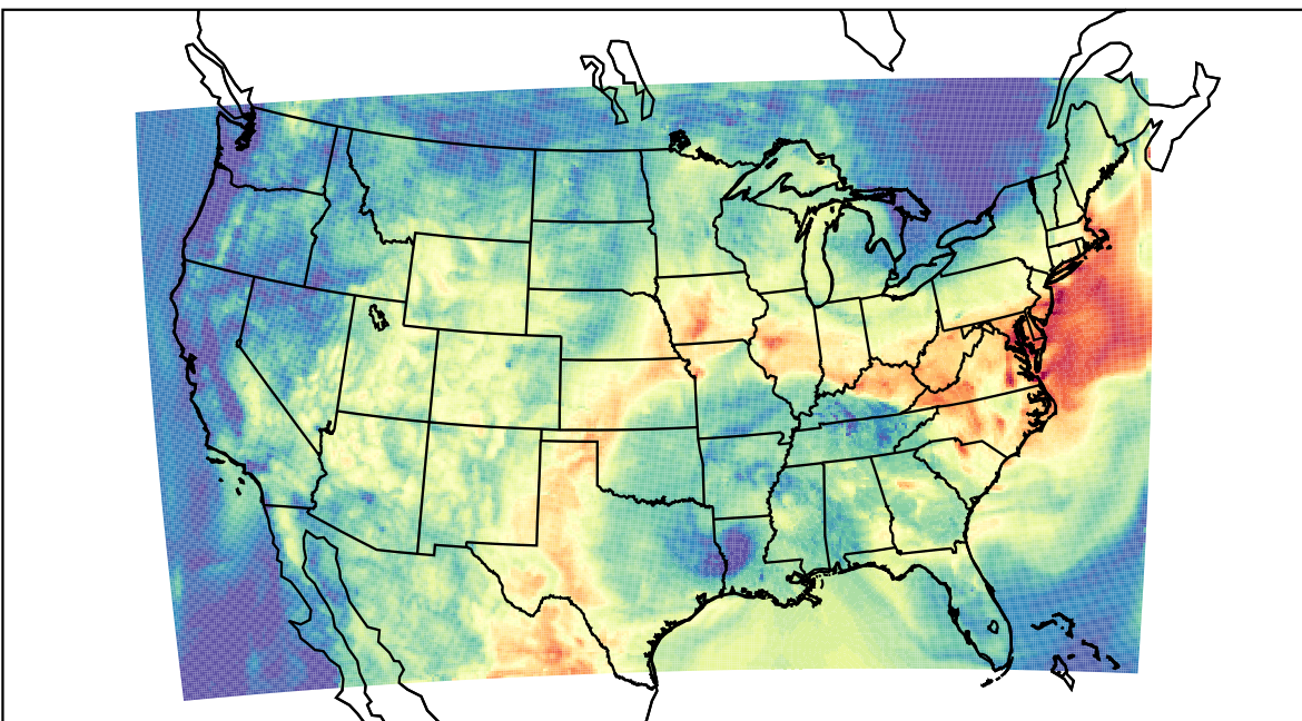
WRF (2019-07-14_15:00:00)
