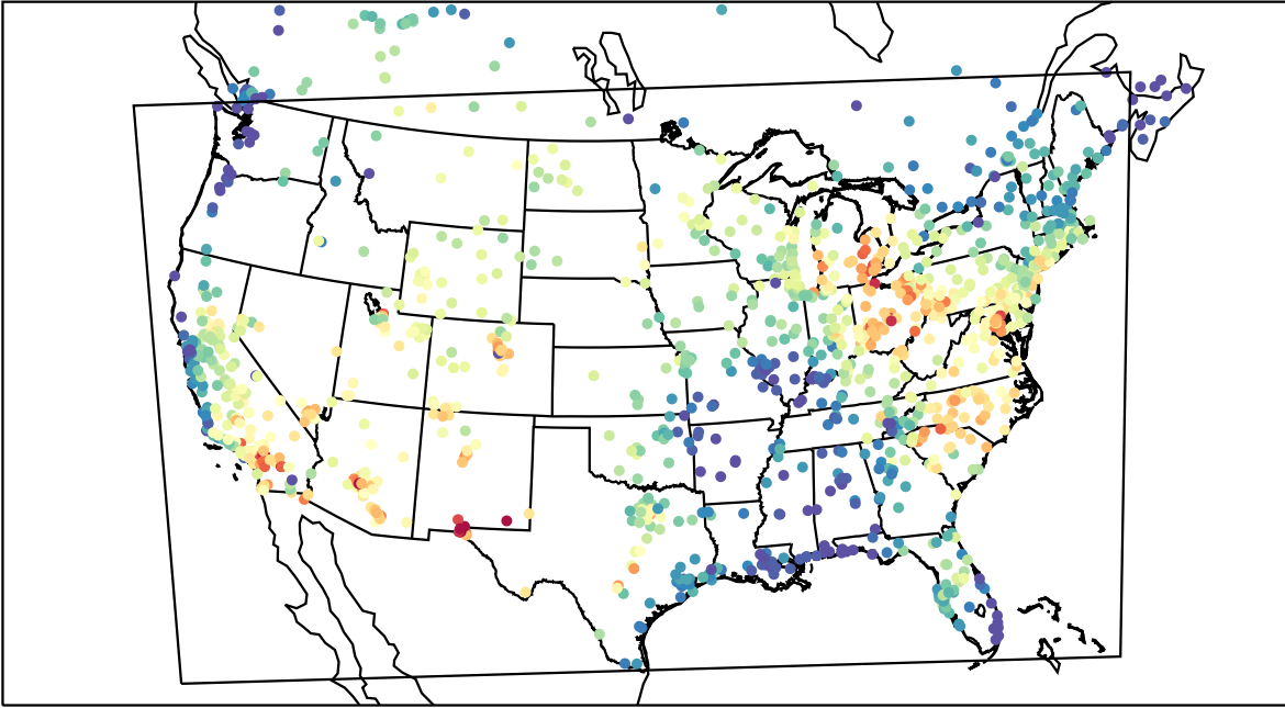
AirNOW (2019-07-15_18:00:00)
