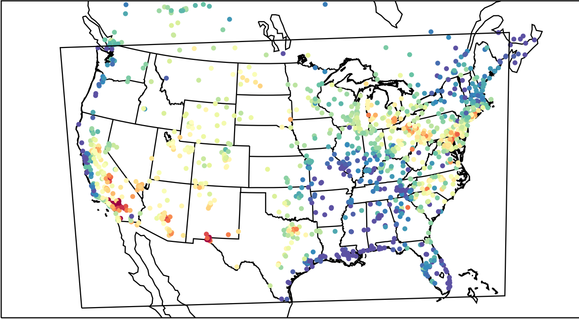
AirNOW (2019-07-15_23:00:00)
