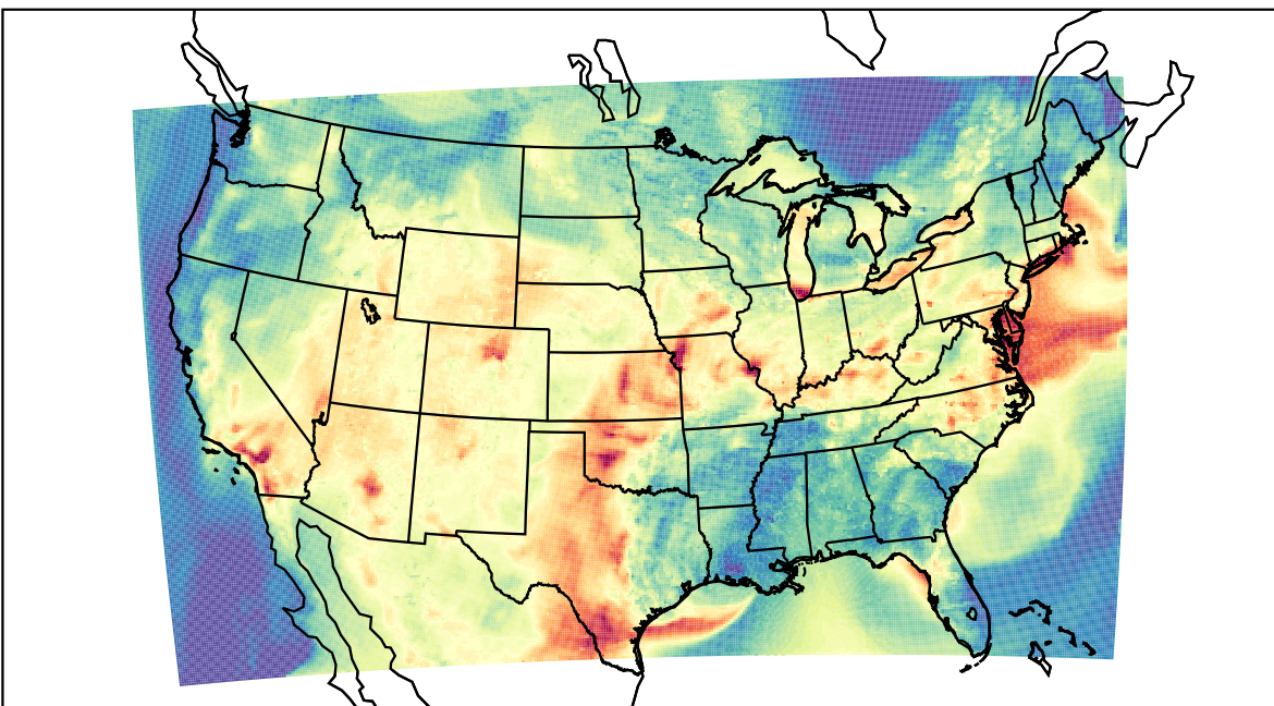
WRF (2019-07-14_00:00:00)
