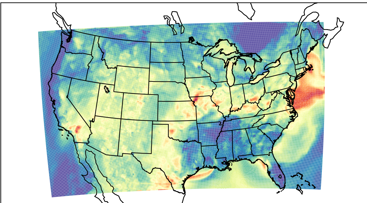
WRF (2019-07-14_03:00:00)
