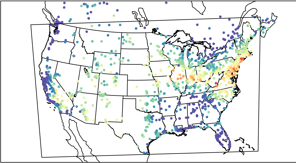
AirNOW (2019-07-14_15:00:00)
