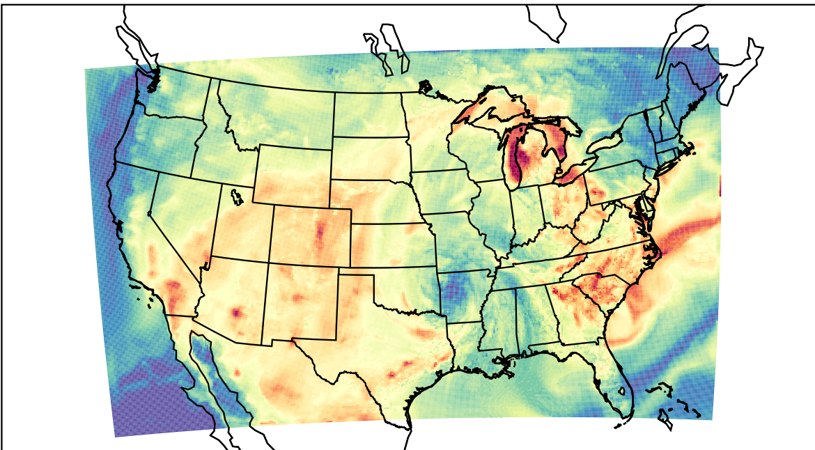
WRF (2019-07-15_23:00:00)
