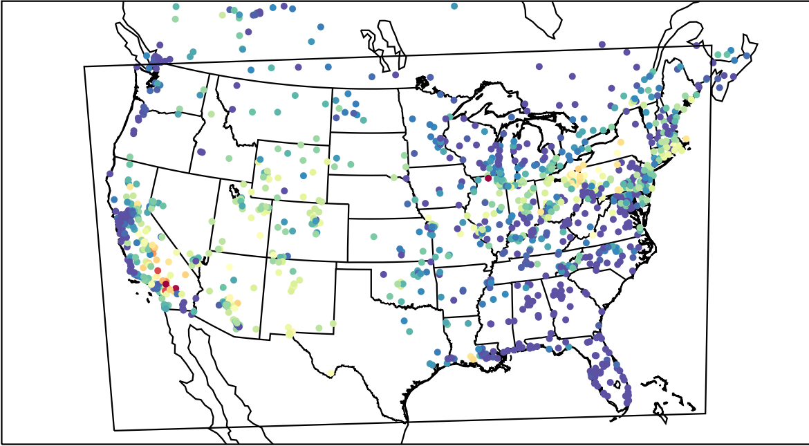
AirNOW (2019-07-14_04:00:00)
