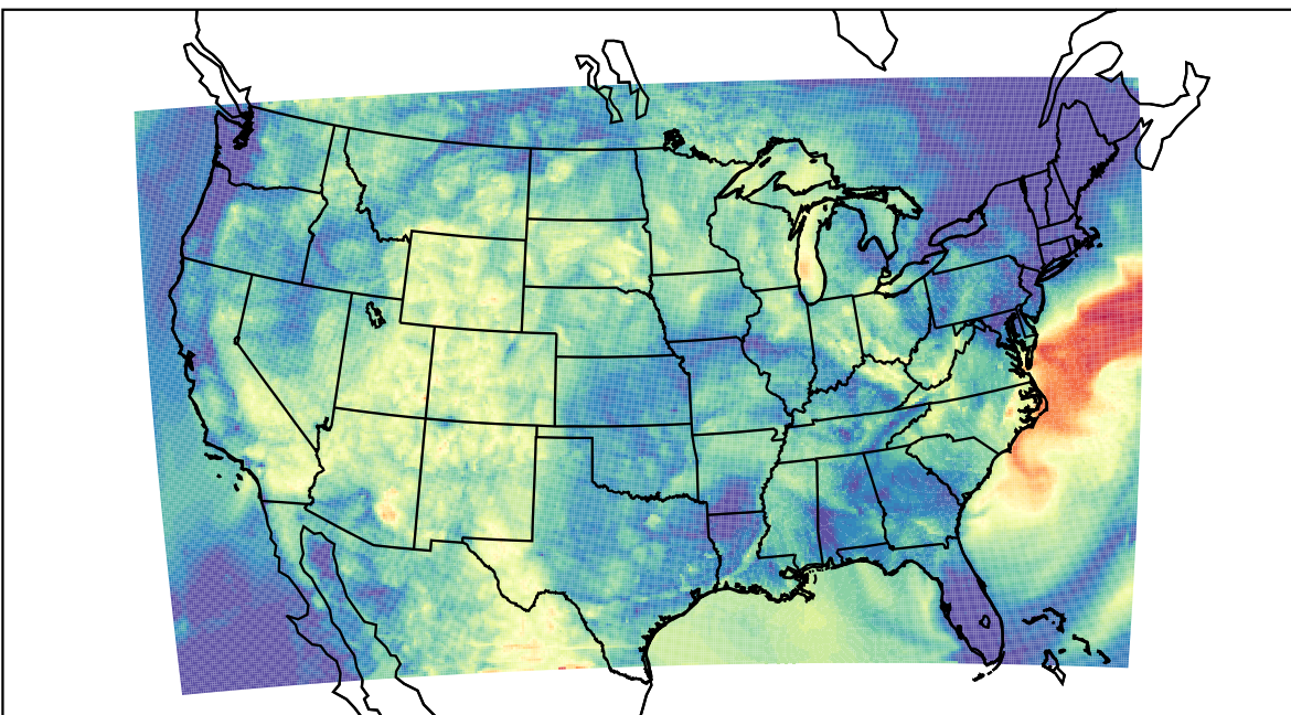
WRF (2019-07-15_07:00:00)
