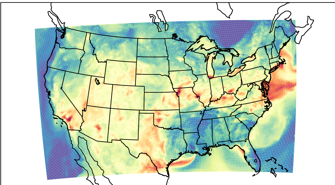
WRF (2019-07-14_01:00:00)
