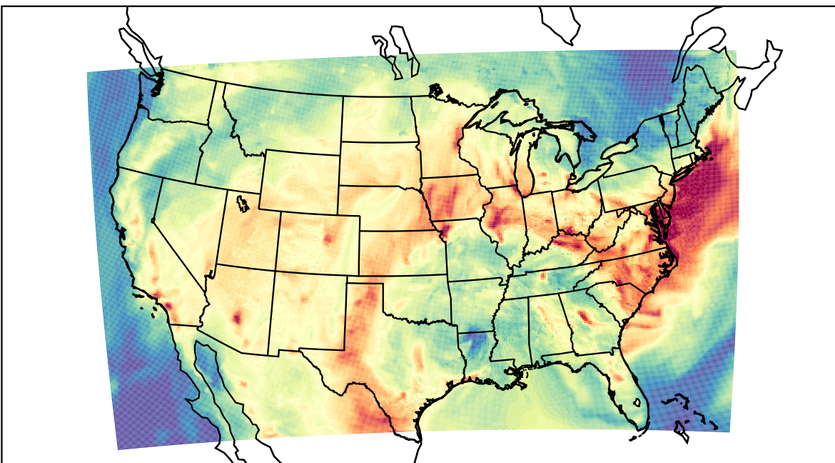
WRF (2019-07-14_21:00:00)
