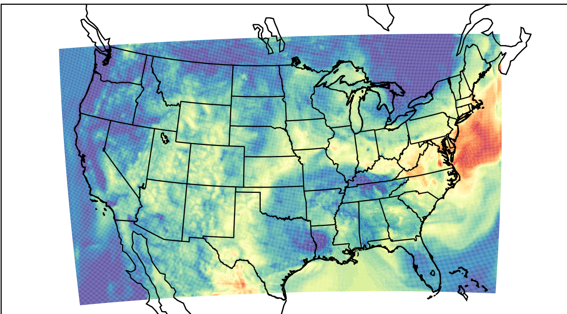
WRF (2019-07-14_14:00:00)
