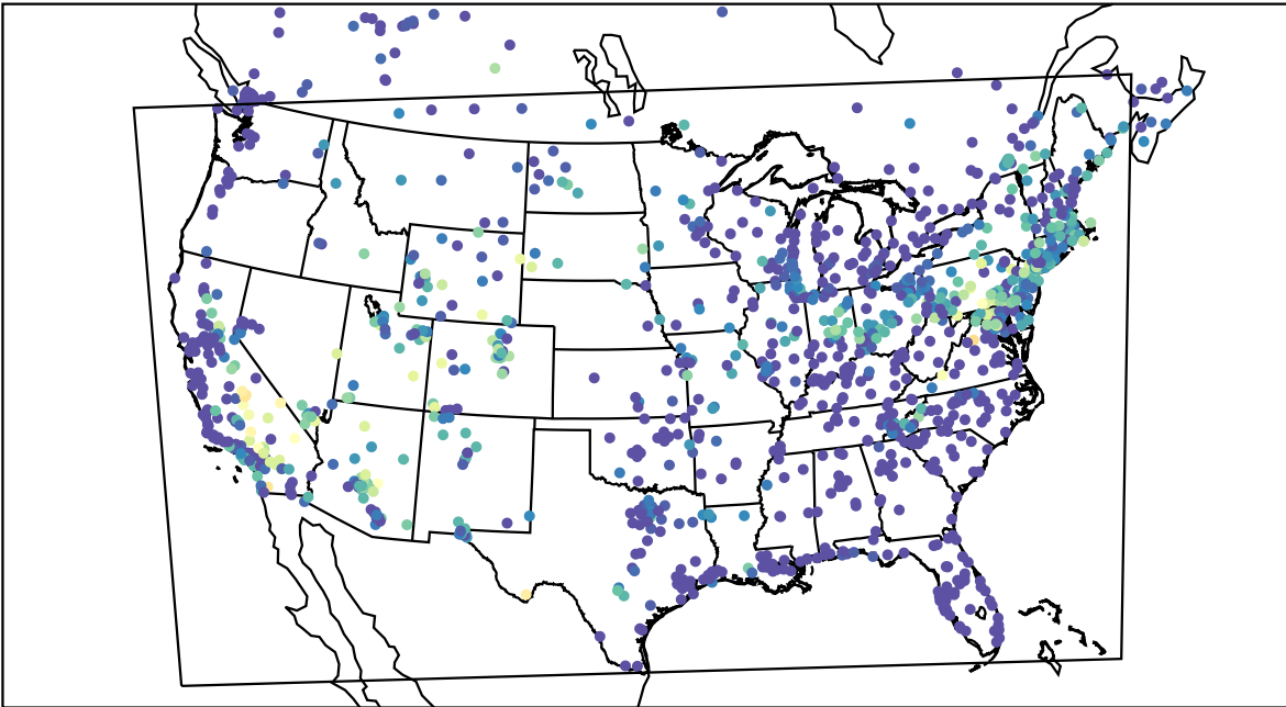
AirNOW (2019-07-14_11:00:00)
