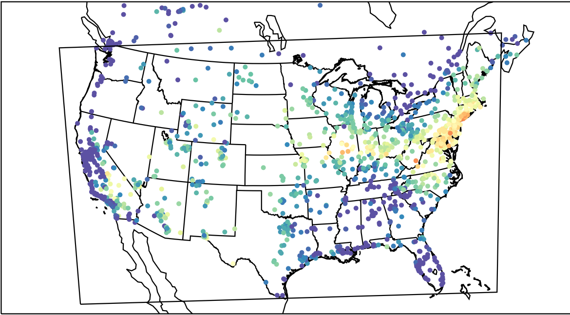
AirNOW (2019-07-14_14:00:00)
