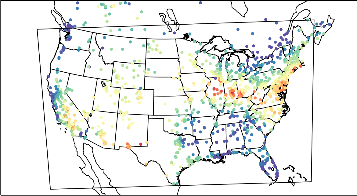
AirNOW (2019-07-14_17:00:00)
