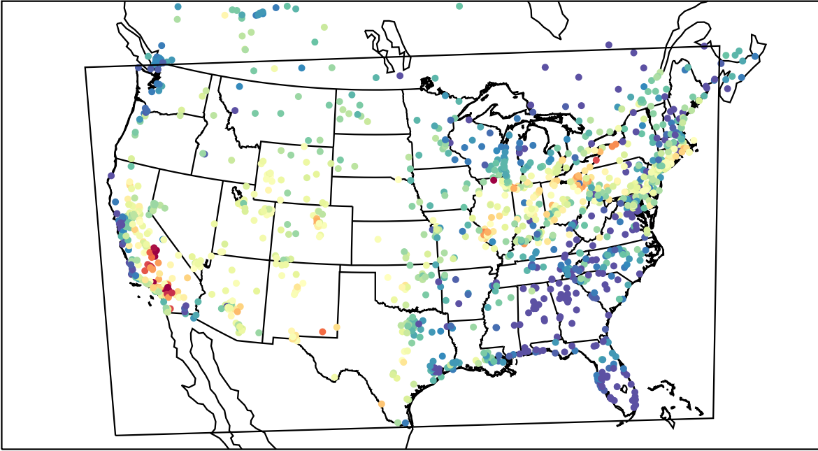
AirNOW (2019-07-14_01:00:00)
