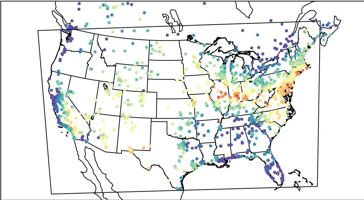
AirNOW (2019-07-14_16:00:00)
