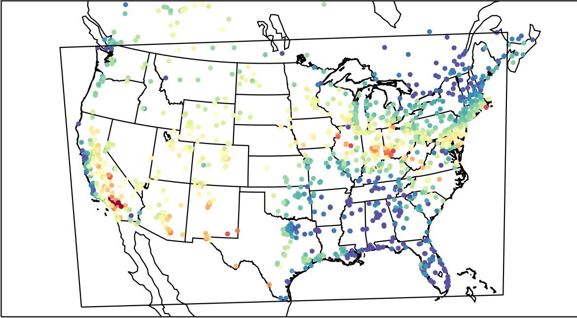
AirNOW (2019-07-14_23:00:00)
