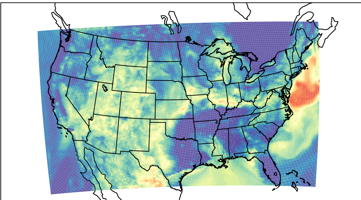
WRF (2019-07-14_10:00:00)
