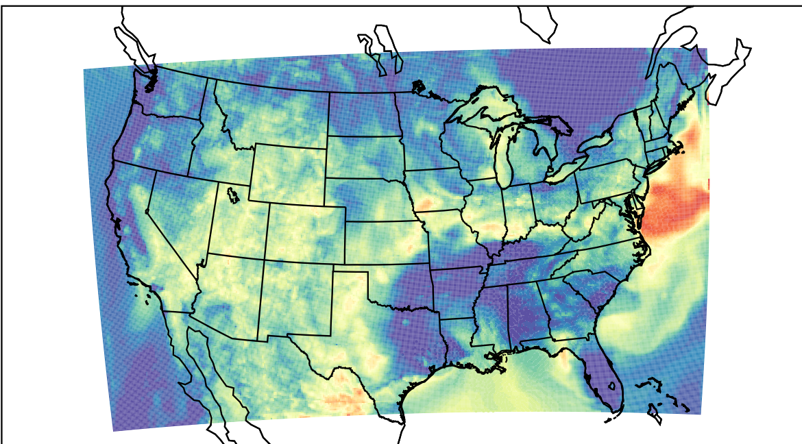
WRF (2019-07-14_08:00:00)
