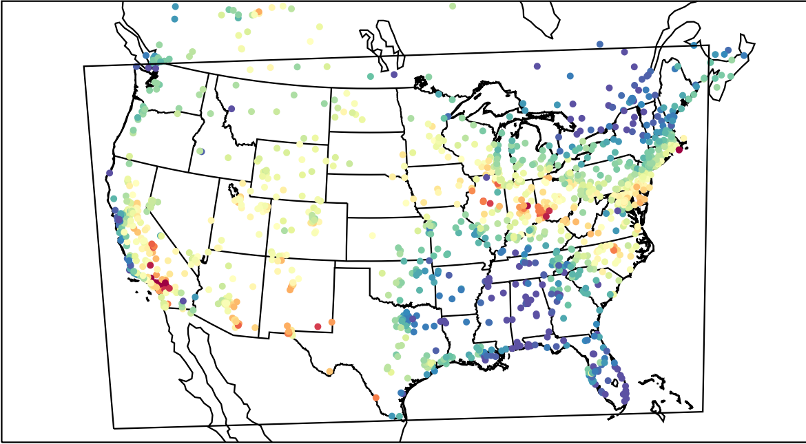
AirNOW (2019-07-14_22:00:00)
