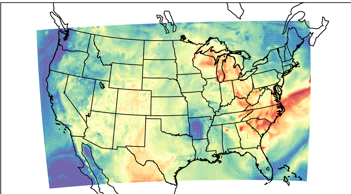
WRF (2019-07-15_16:00:00)
