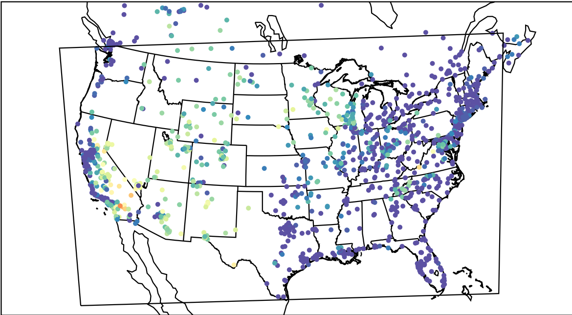
AirNOW (2019-07-15_06:00:00)
