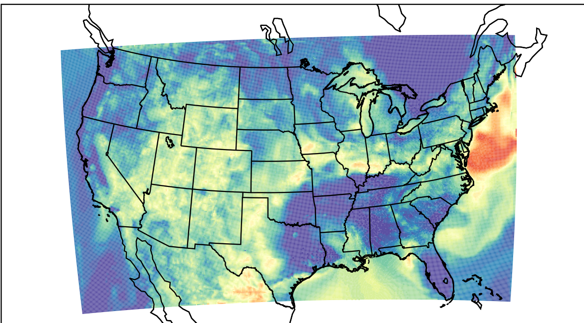
WRF (2019-07-14_09:00:00)
