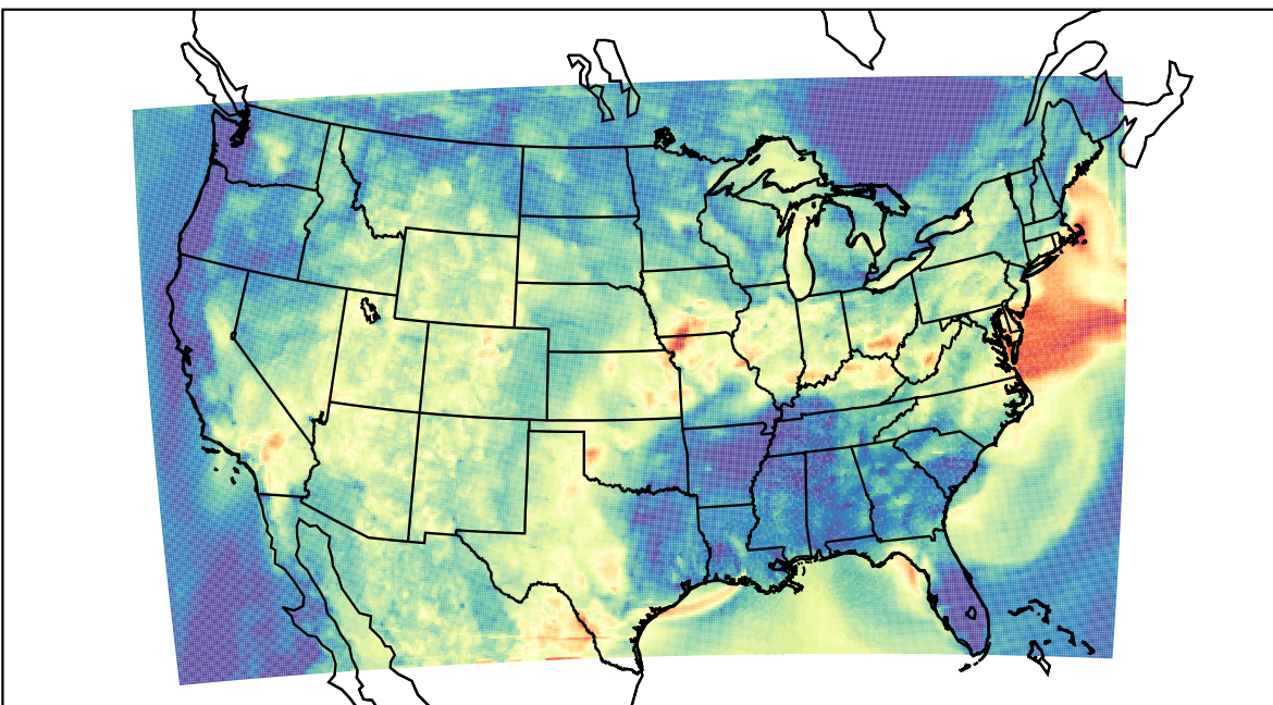
WRF (2019-07-14_04:00:00)
