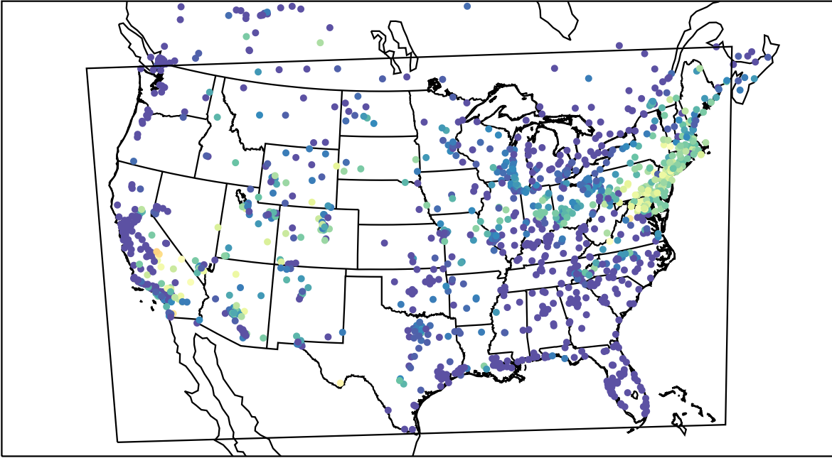
AirNOW (2019-07-14_12:00:00)
