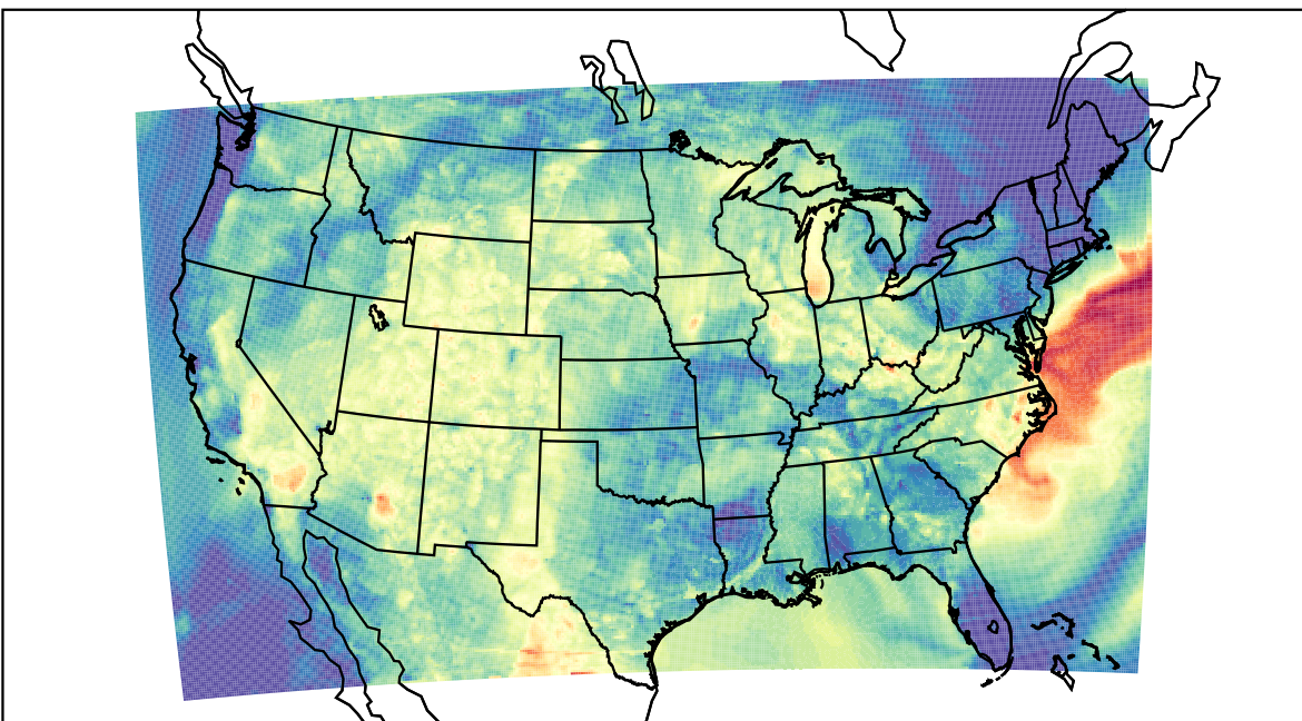
WRF (2019-07-15_04:00:00)
