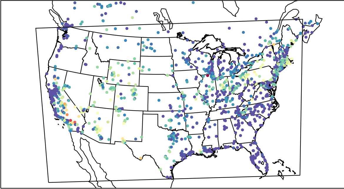
AirNOW (2019-07-14_06:00:00)
