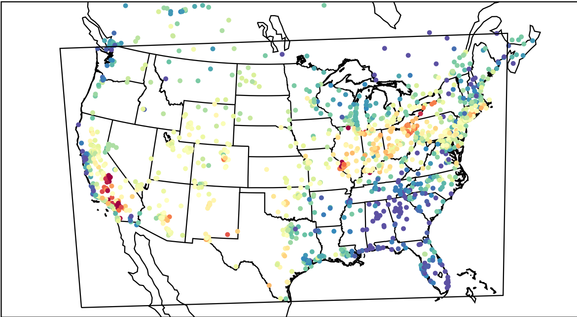
AirNOW (2019-07-14_00:00:00)
