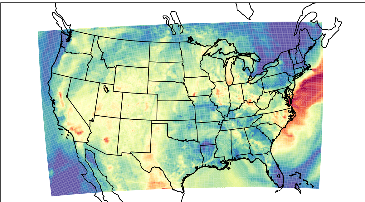
WRF (2019-07-15_02:00:00)
