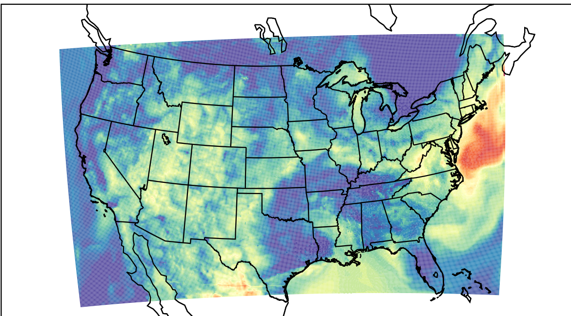
WRF (2019-07-14_13:00:00)
