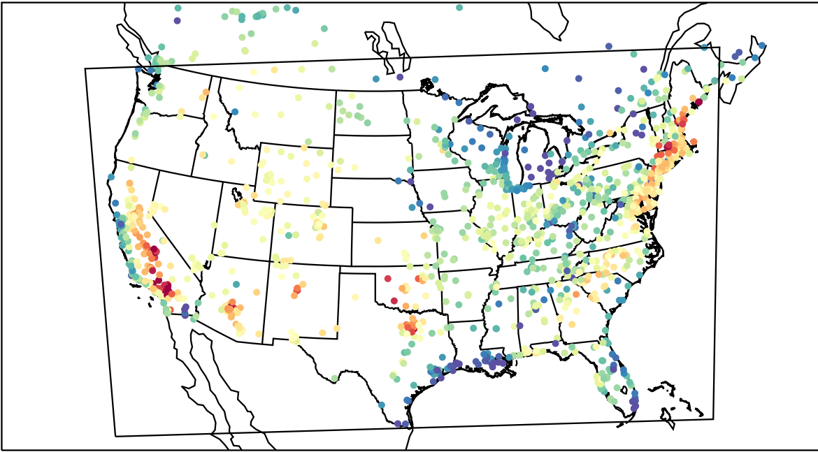
AirNOW (2019-07-30_23:00:00)
