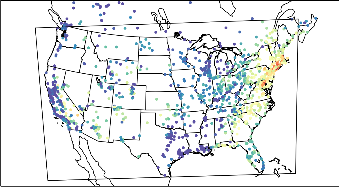
AirNOW (2019-07-30_14:00:00)
