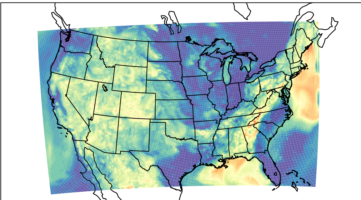
WRF (2019-07-31_09:00:00)
