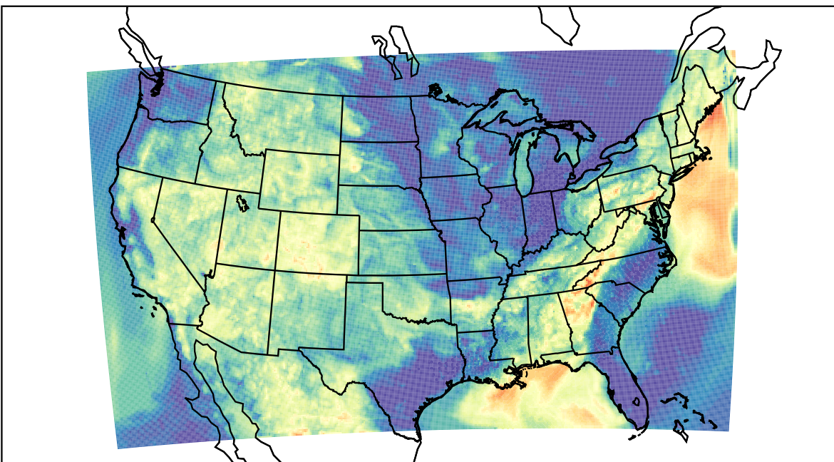
WRF (2019-07-31_08:00:00)
