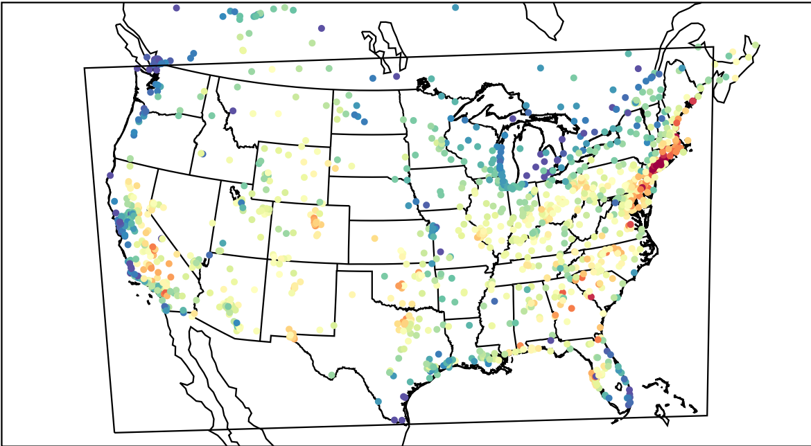
AirNOW (2019-07-31_17:00:00)
