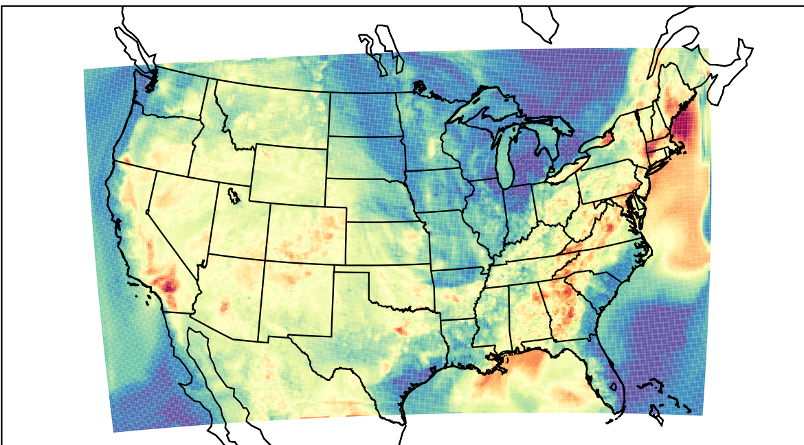
WRF (2019-07-31_02:00:00)
