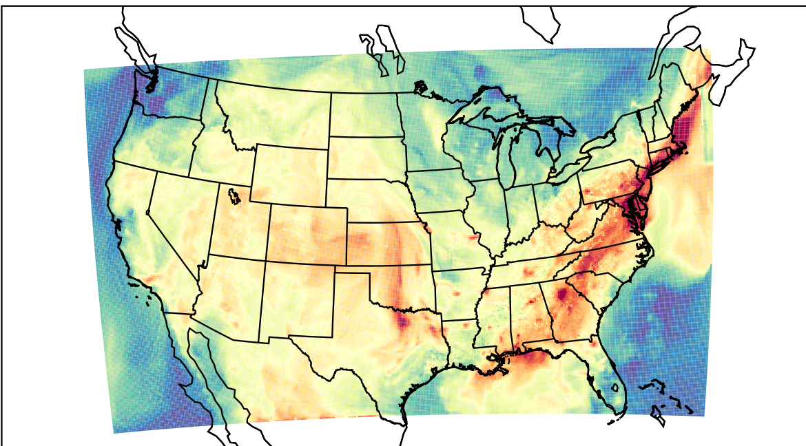
WRF (2019-07-31_18:00:00)
