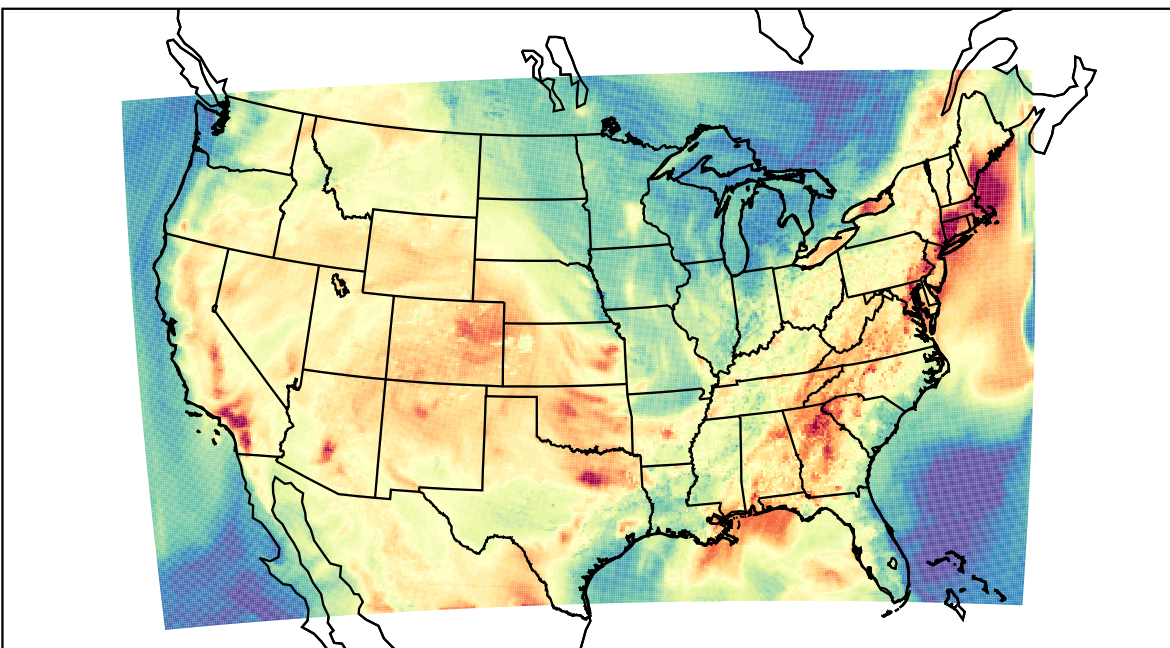
WRF (2019-07-30_23:00:00)
