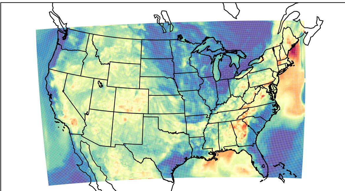
WRF (2019-07-31_04:00:00)
