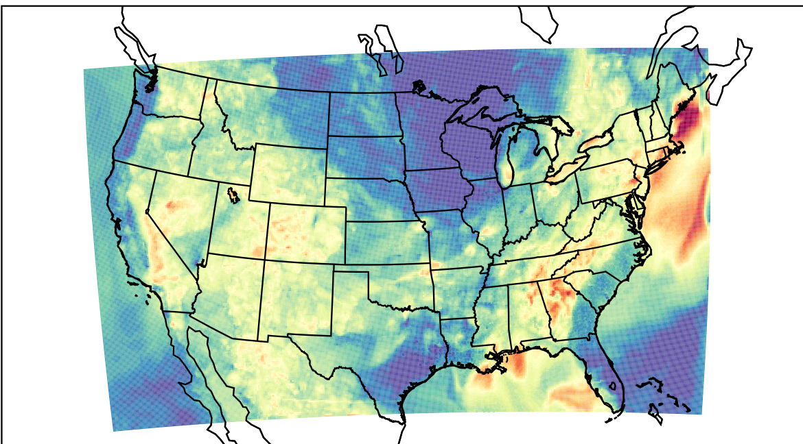
WRF (2019-07-30_04:00:00)
