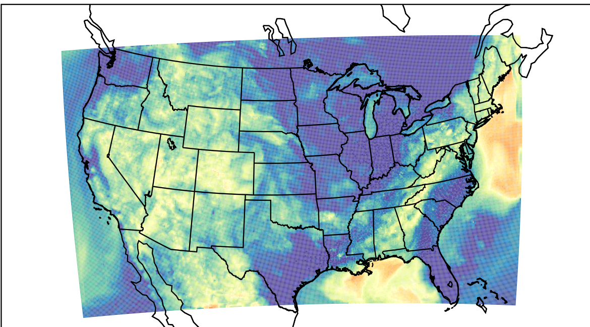
WRF (2019-07-31_12:00:00)
