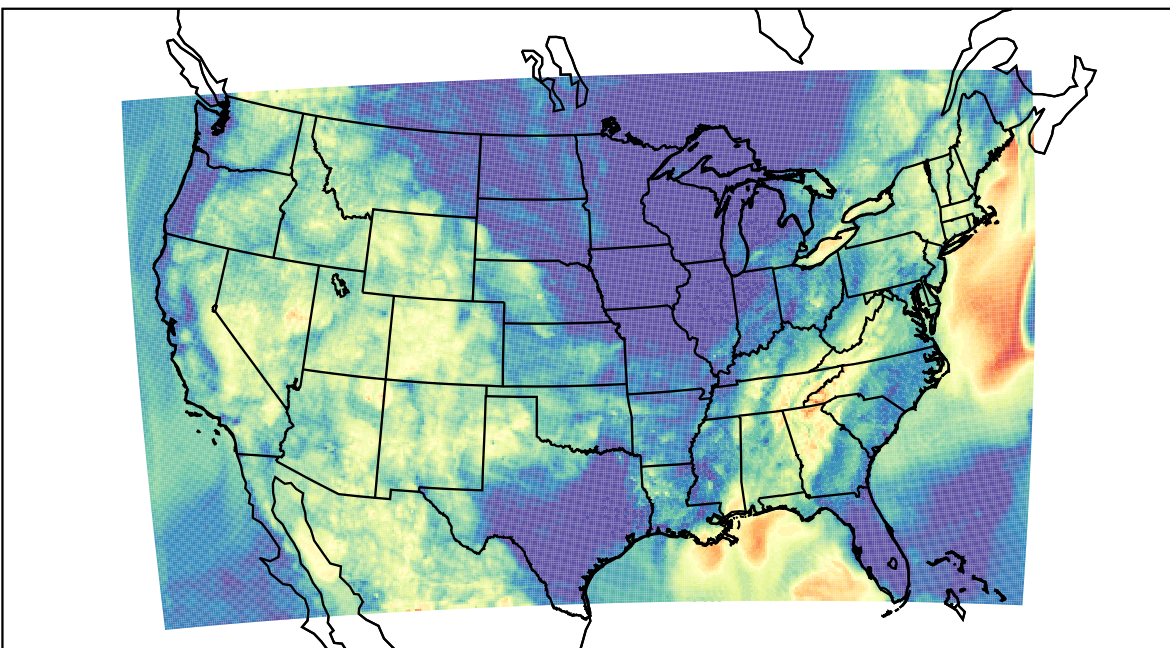
WRF (2019-07-30_11:00:00)
