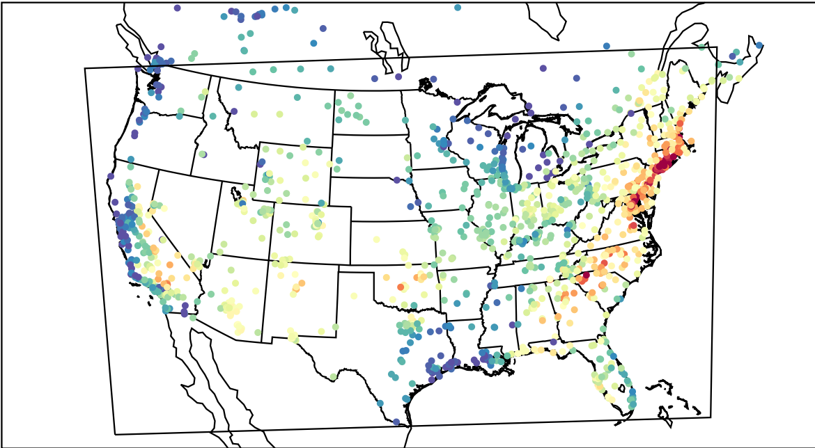
AirNOW (2019-07-30_16:00:00)
