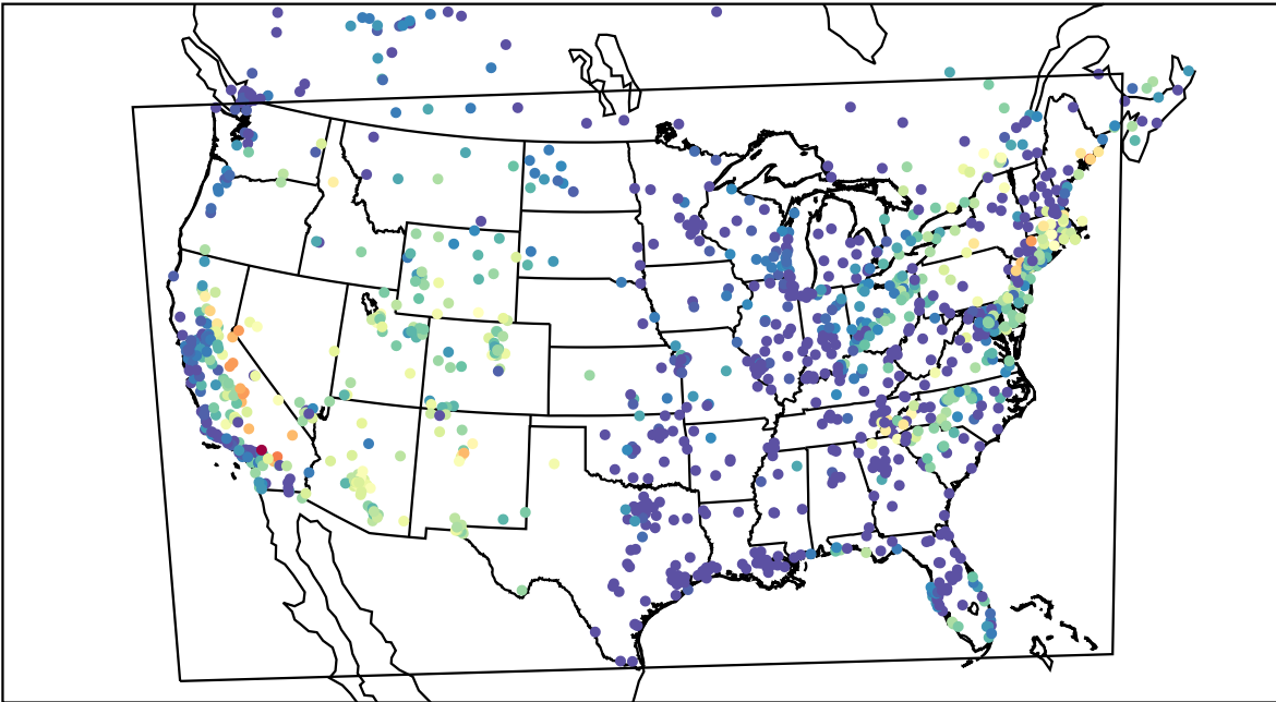
AirNOW (2019-07-30_06:00:00)
