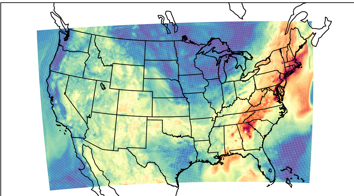
WRF (2019-07-30_15:00:00)
