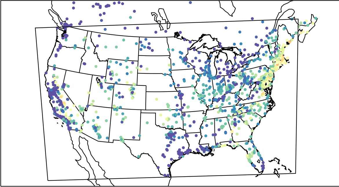
AirNOW (2019-07-31_14:00:00)
