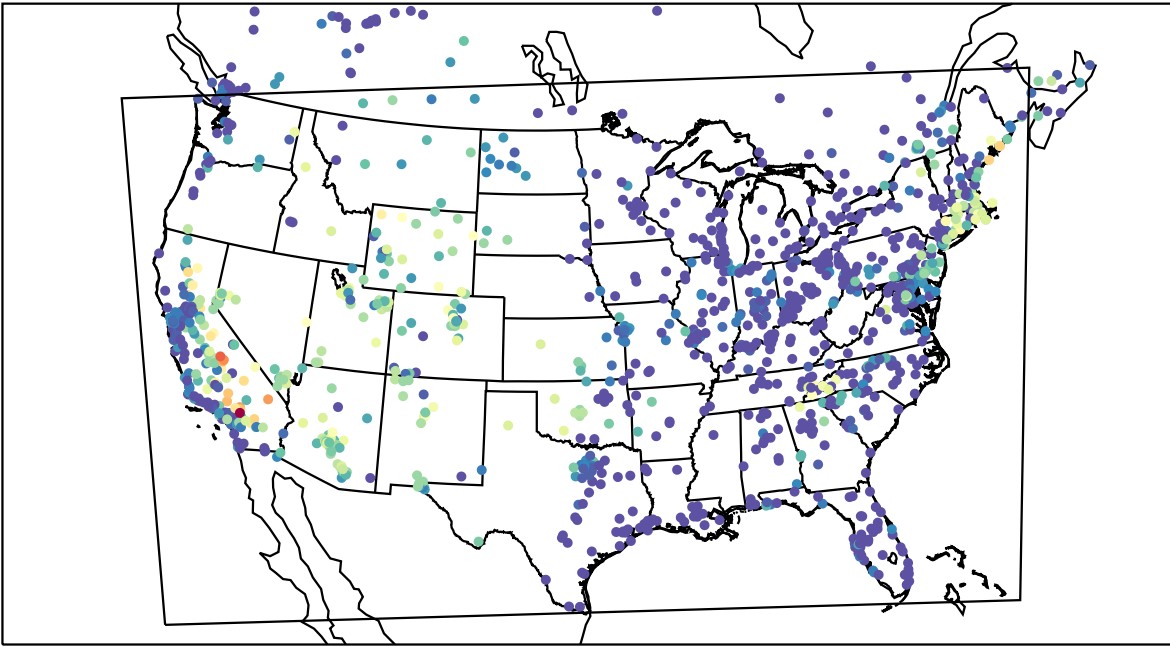
AirNOW (2019-07-31_07:00:00)
