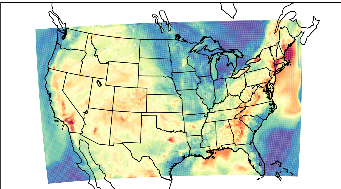
WRF (2019-07-31_01:00:00)
