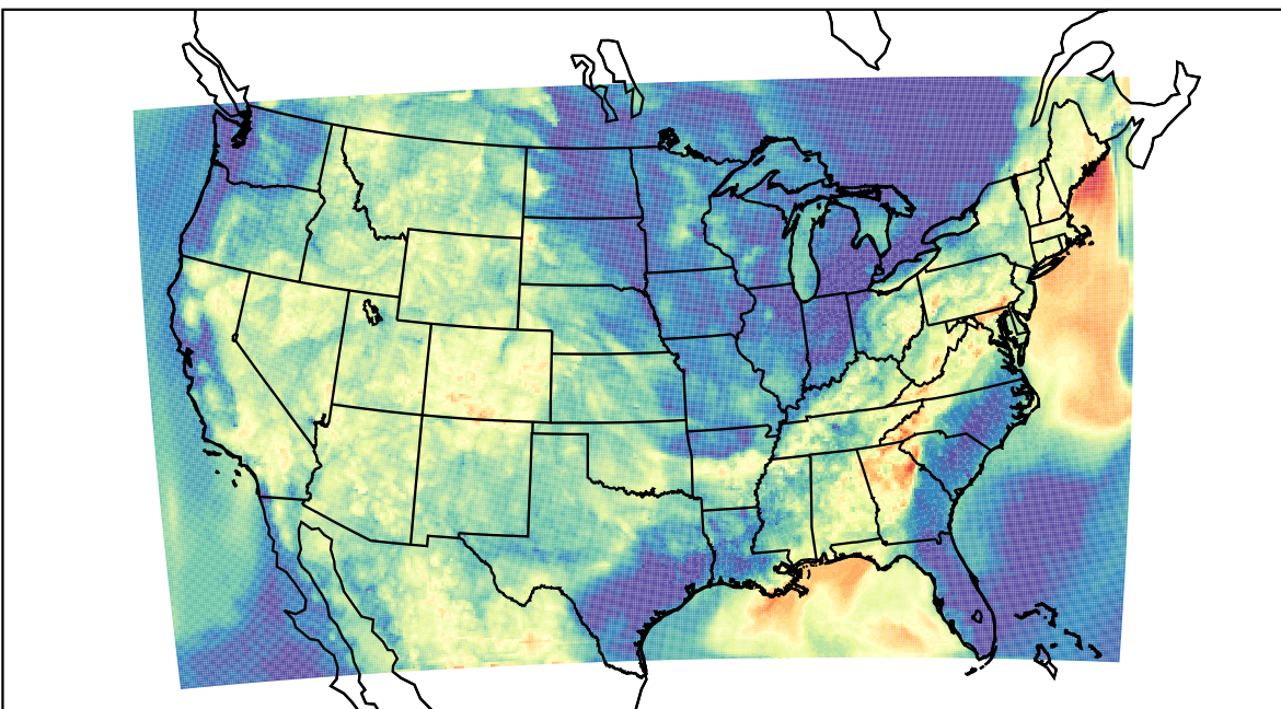
WRF (2019-07-31_06:00:00)
