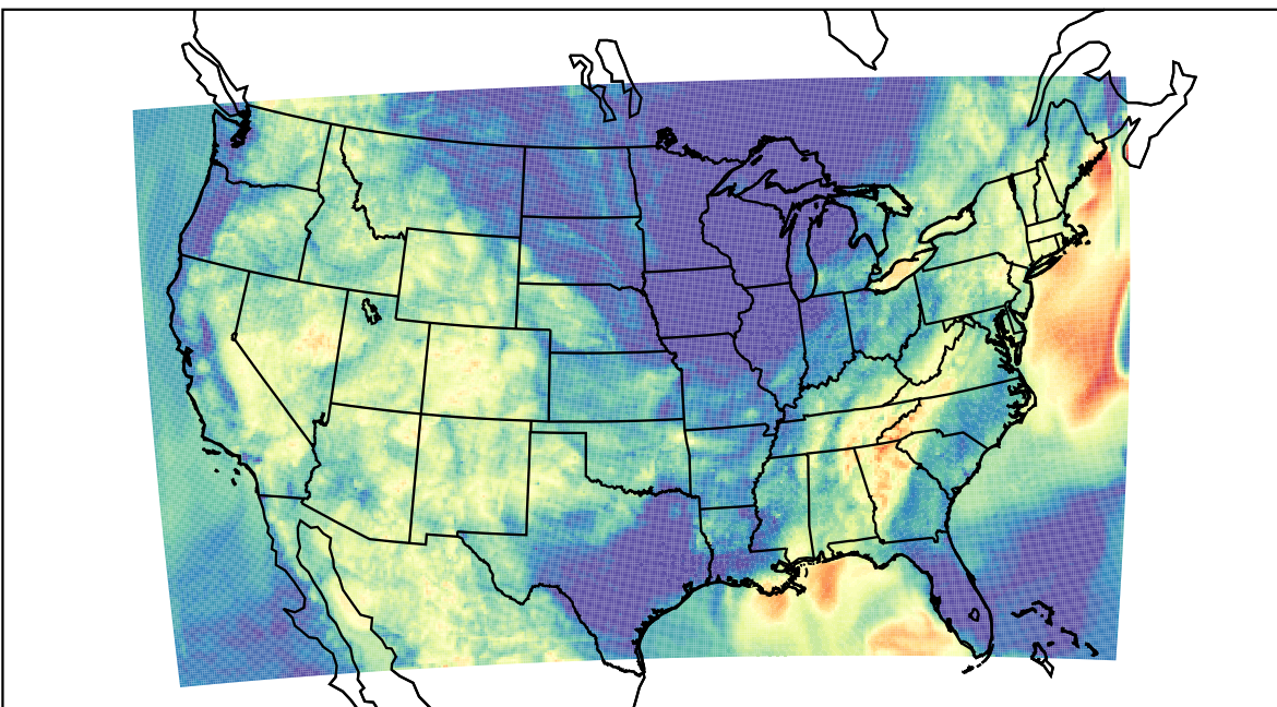
WRF (2019-07-30_09:00:00)
