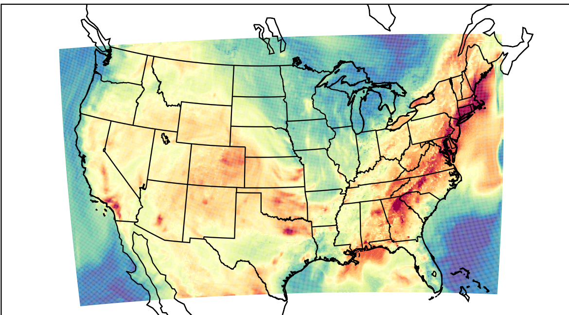
WRF (2019-07-30_21:00:00)
