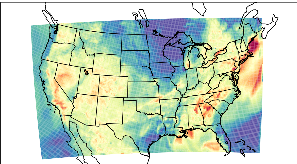
WRF (2019-07-30_02:00:00)
