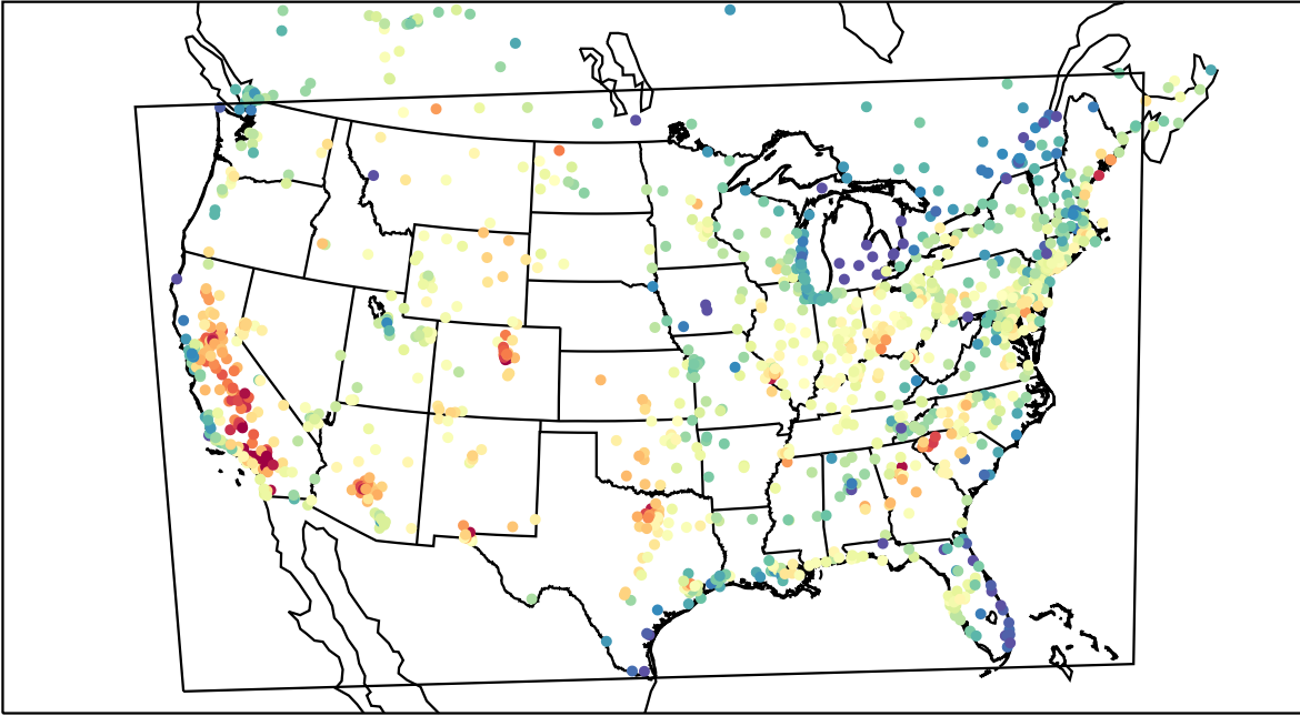
AirNOW (2019-07-31_22:00:00)
