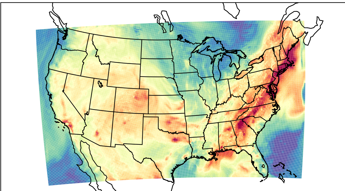
WRF (2019-07-30_20:00:00)
