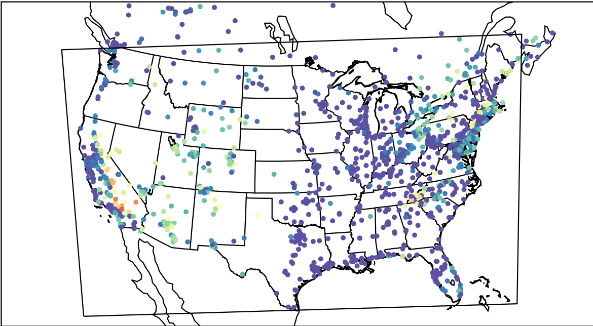
AirNOW (2019-07-30_09:00:00)
