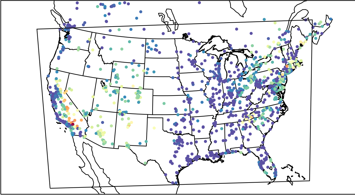
AirNOW (2019-07-30_07:00:00)
