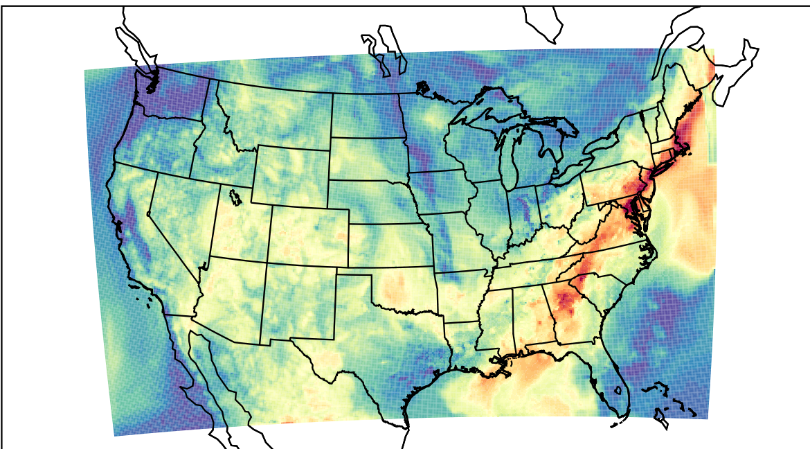
WRF (2019-07-31_15:00:00)
