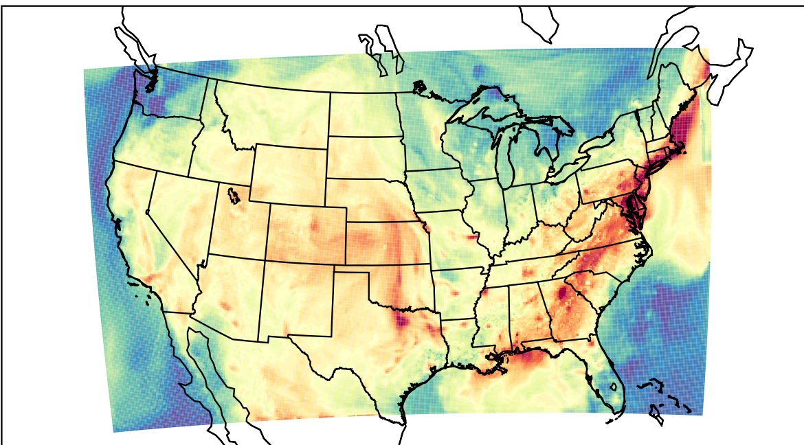
WRF (2019-07-31_19:00:00)
