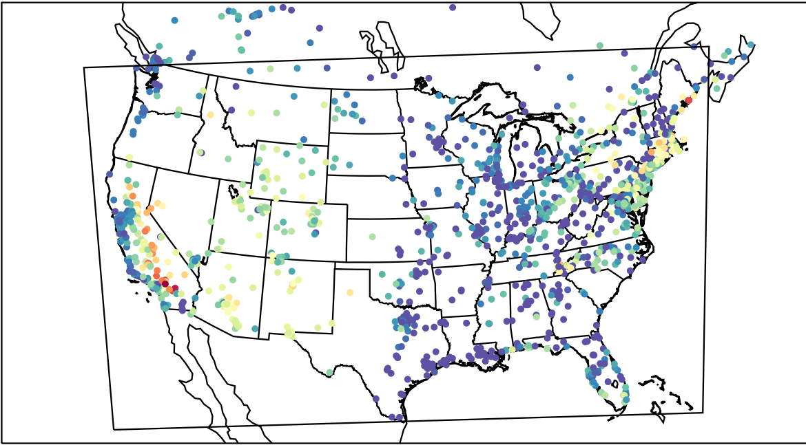
AirNOW (2019-07-30_04:00:00)
