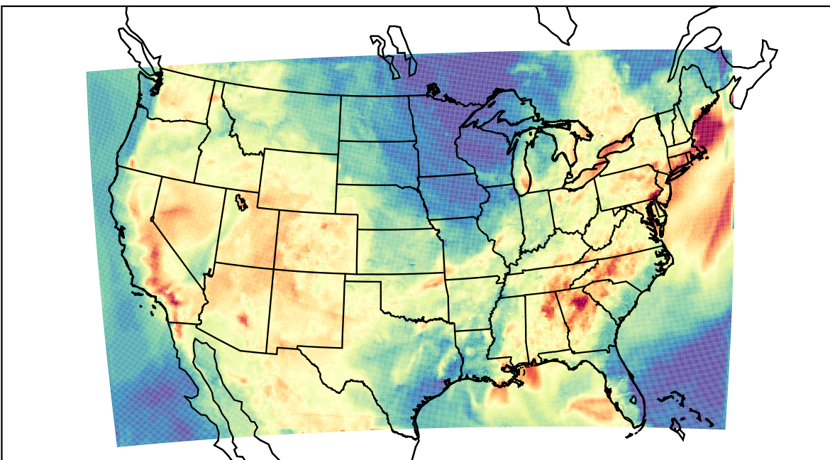
WRF (2019-07-30_01:00:00)
