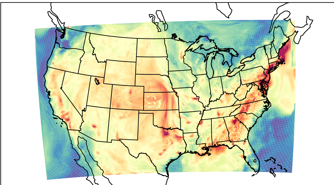
WRF (2019-07-31_22:00:00)
