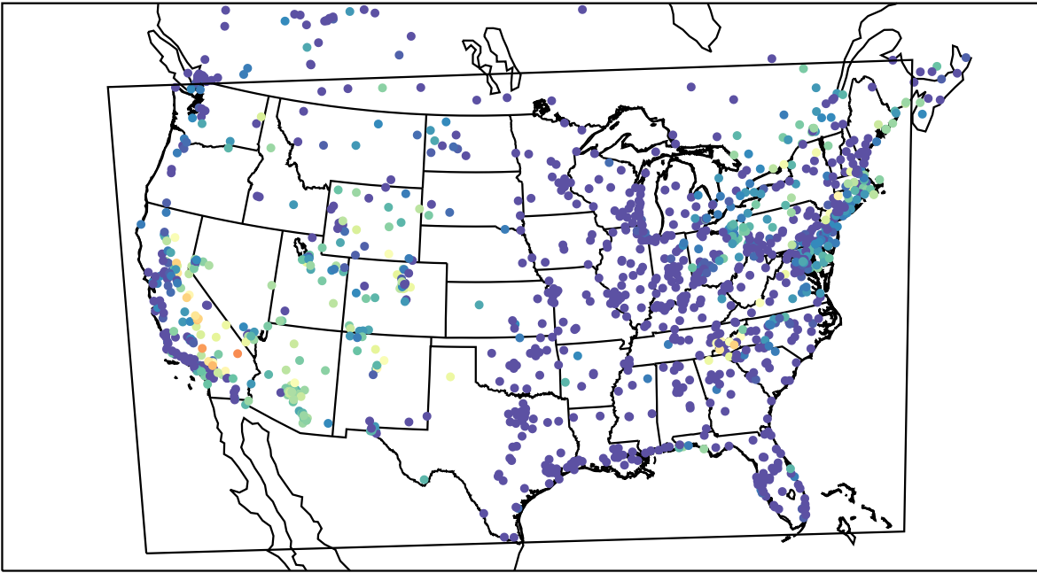
AirNOW (2019-07-30_11:00:00)
