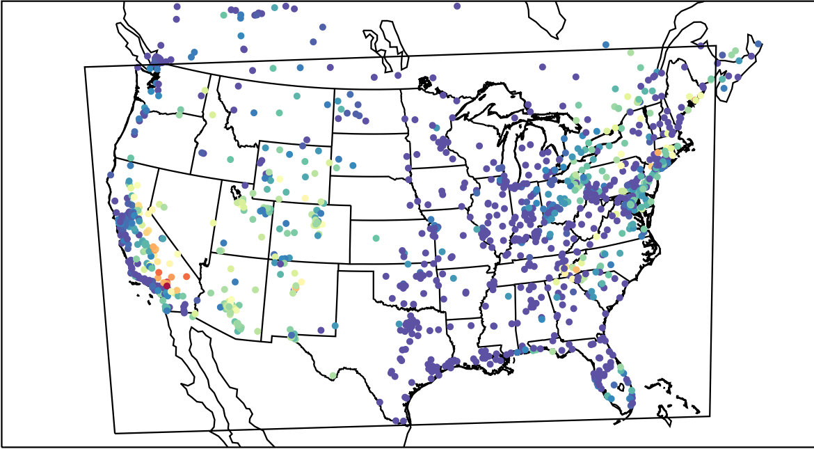
AirNOW (2019-07-30_08:00:00)
