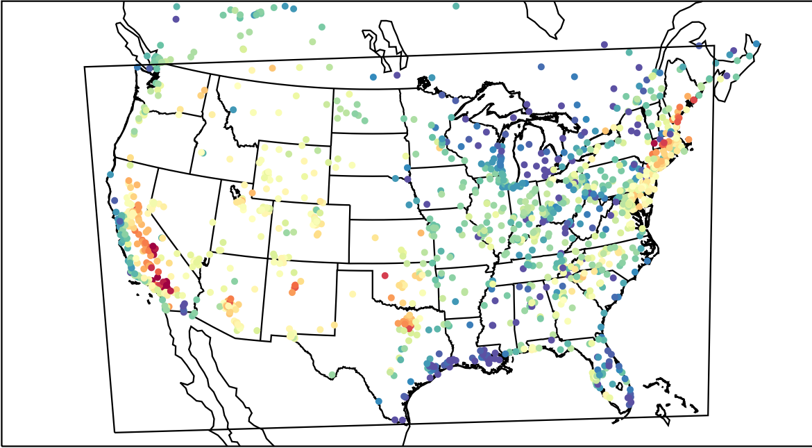
AirNOW (2019-07-31_00:00:00)
