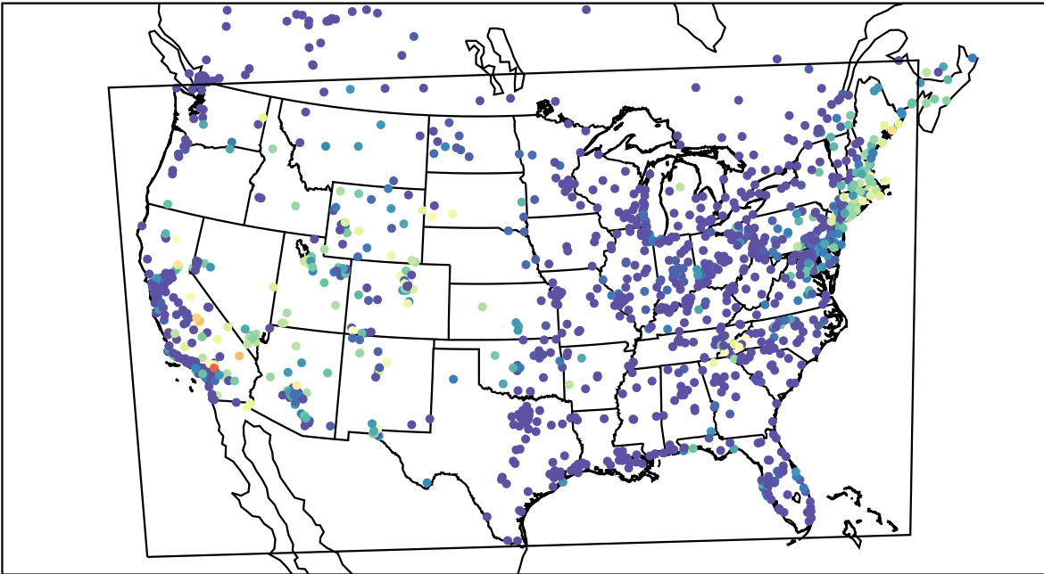
AirNOW (2019-07-31_12:00:00)
