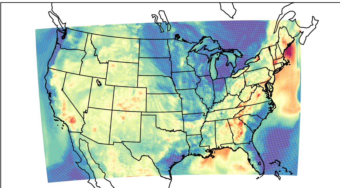
WRF (2019-07-31_03:00:00)
