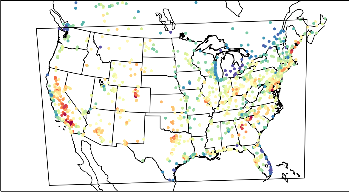
AirNOW (2019-07-31_20:00:00)
