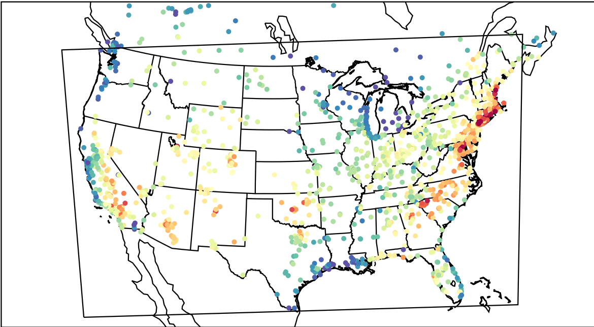
AirNOW (2019-07-30_18:00:00)
