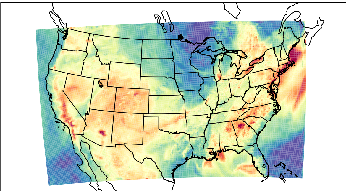
WRF (2019-07-30_00:00:00)
