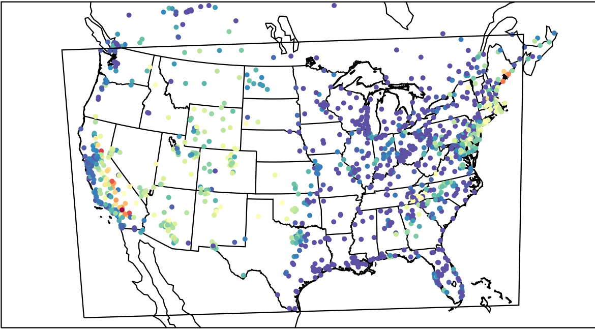
AirNOW (2019-07-31_05:00:00)
