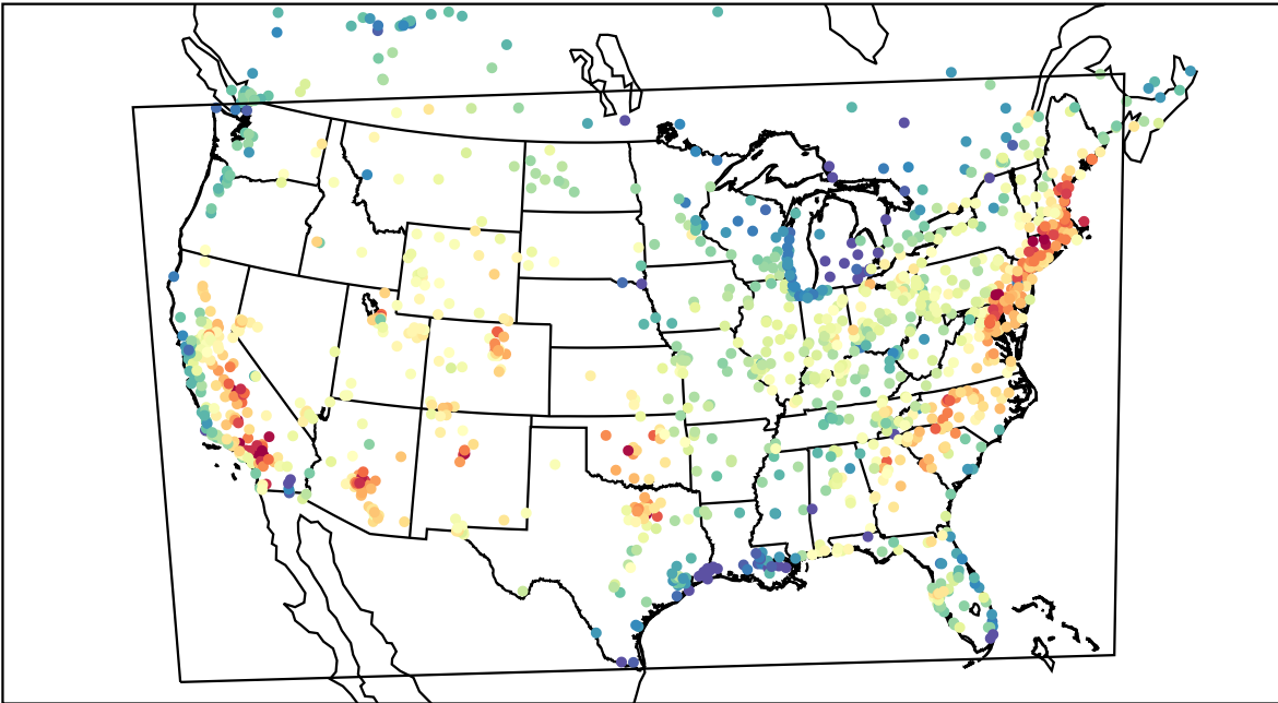
AirNOW (2019-07-30_21:00:00)
