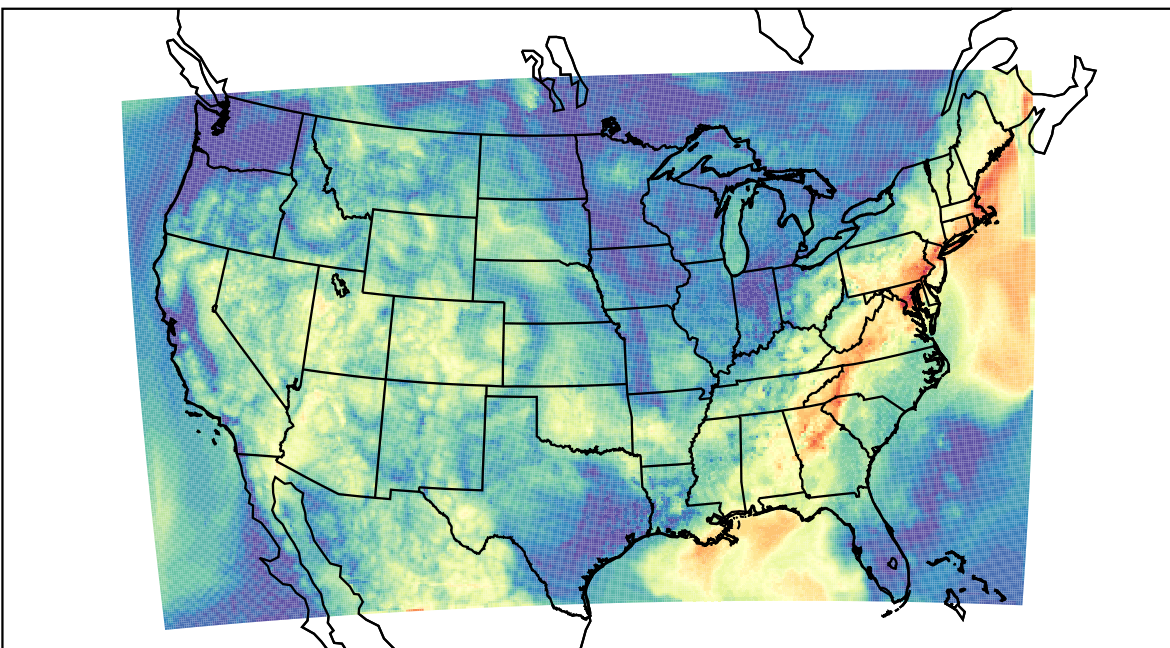
WRF (2019-07-31_14:00:00)
