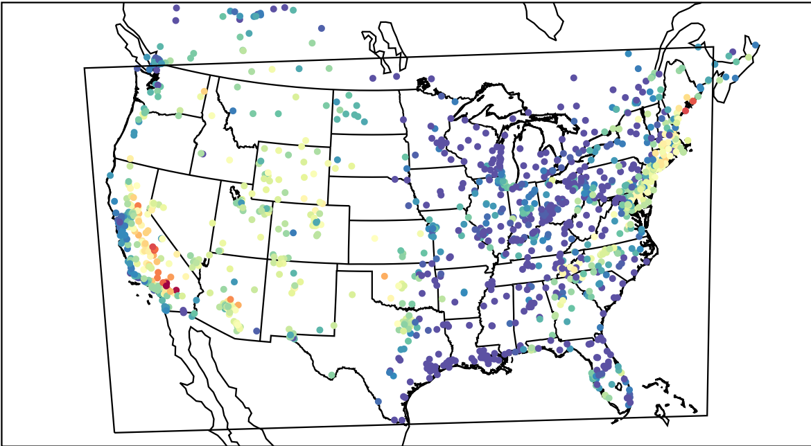
AirNOW (2019-07-31_03:00:00)
