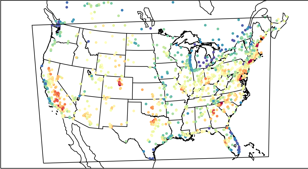
AirNOW (2019-07-31_19:00:00)
