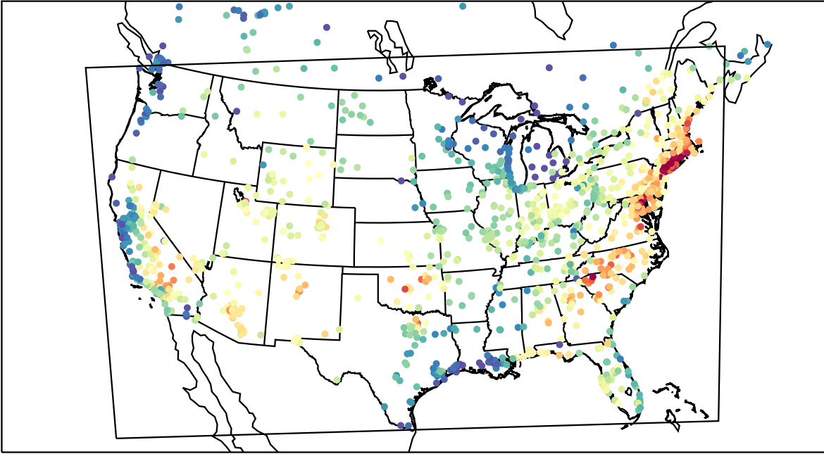
AirNOW (2019-07-30_17:00:00)
