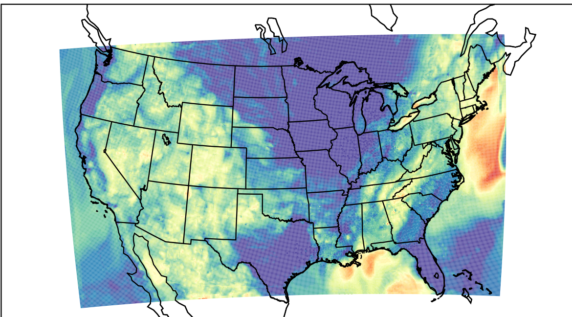
WRF (2019-07-30_12:00:00)
