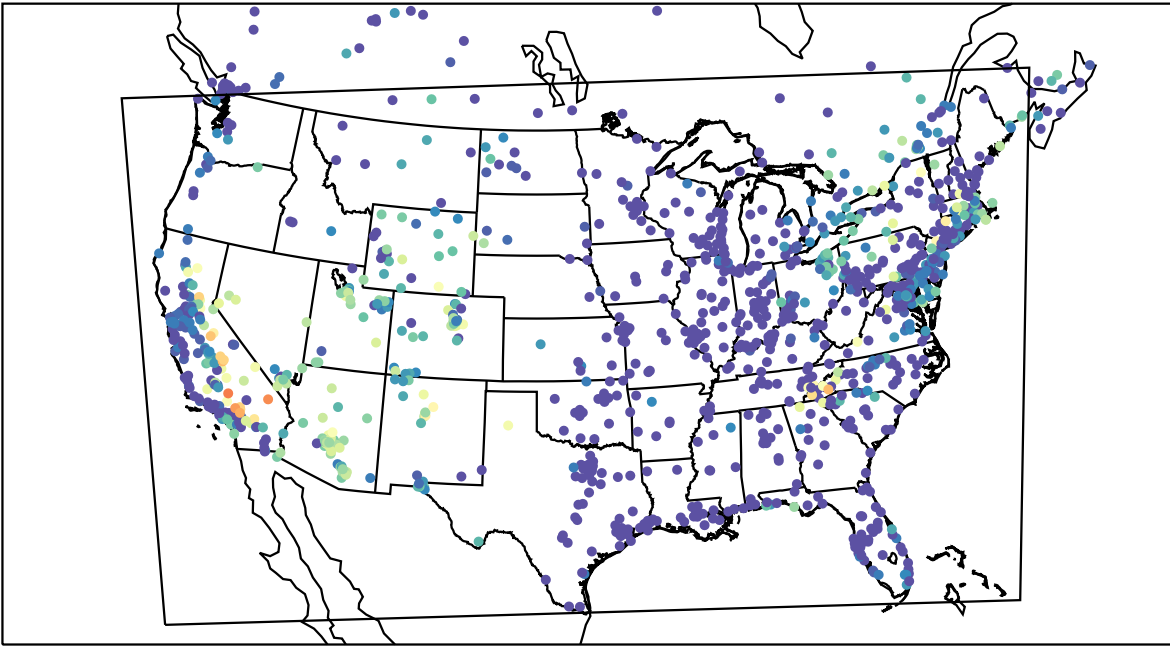
AirNOW (2019-07-30_10:00:00)
