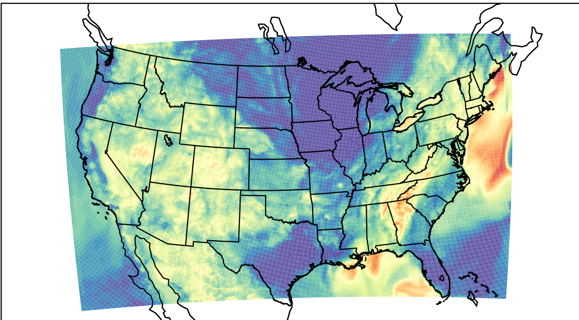
WRF (2019-07-30_08:00:00)
