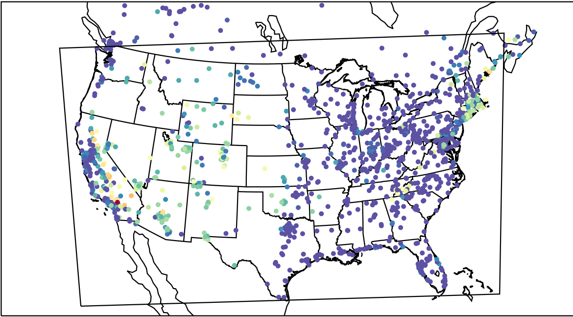
AirNOW (2019-07-31_09:00:00)
