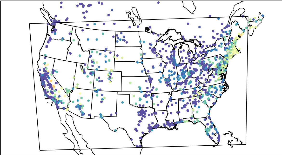
AirNOW (2019-07-31_13:00:00)
