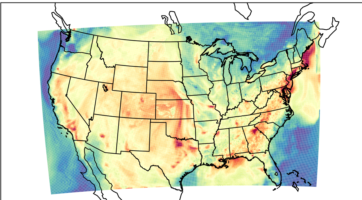
WRF (2019-07-31_23:00:00)
