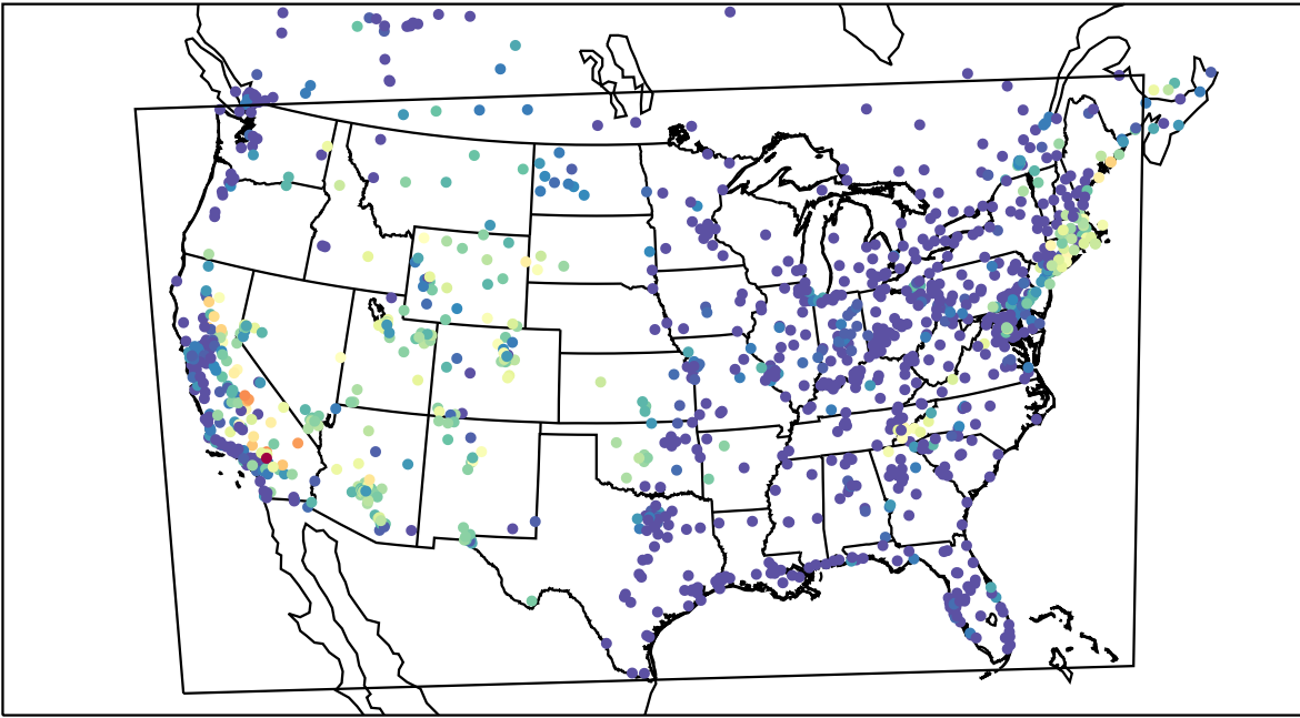
AirNOW (2019-07-31_08:00:00)
