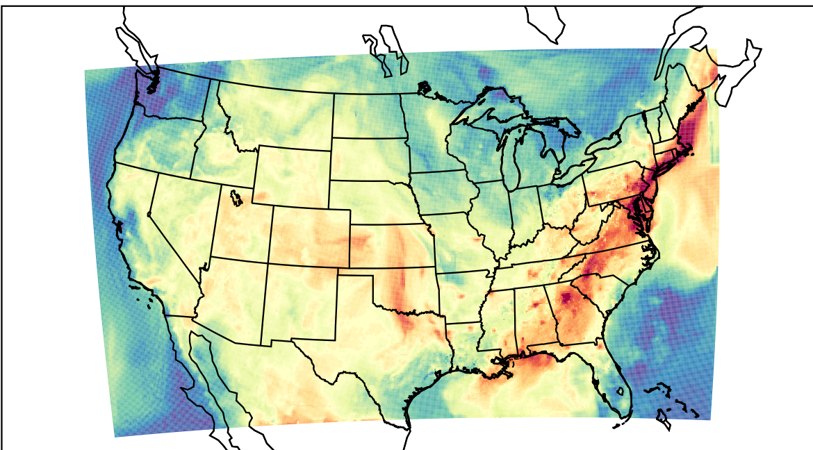
WRF (2019-07-31_17:00:00)
