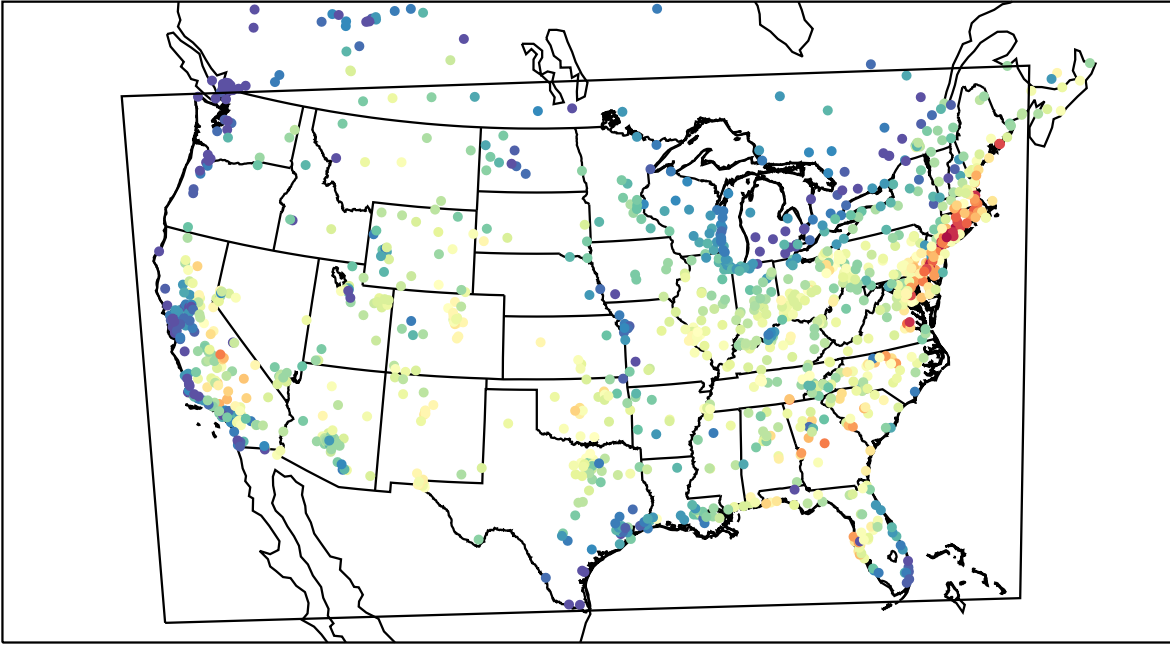
AirNOW (2019-07-31_16:00:00)
