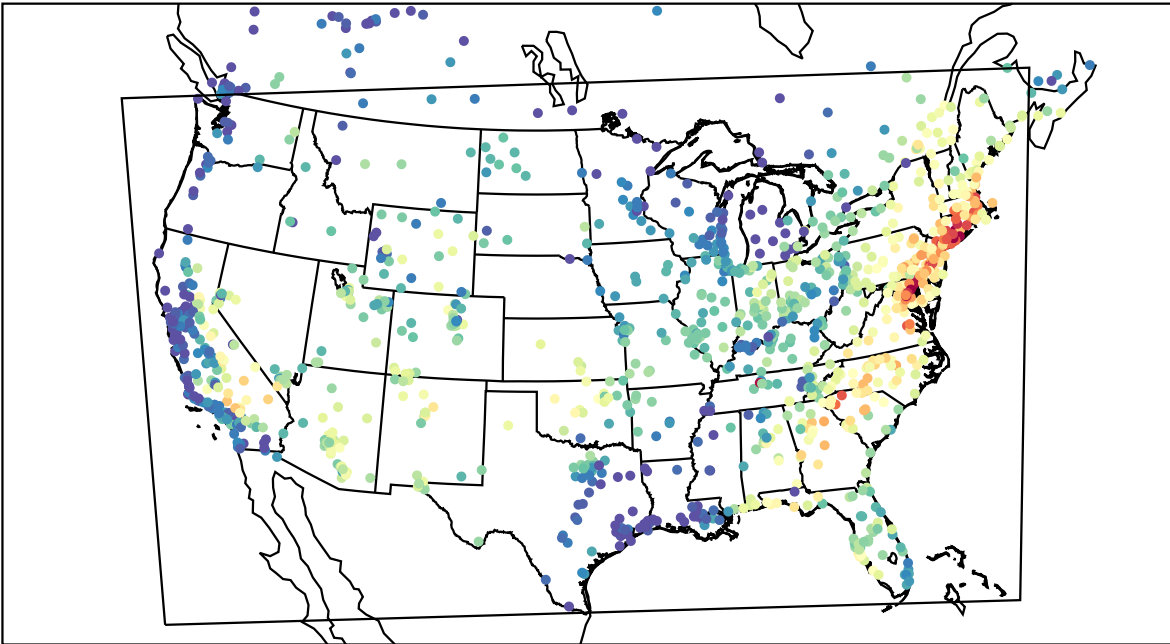
AirNOW (2019-07-30_15:00:00)
