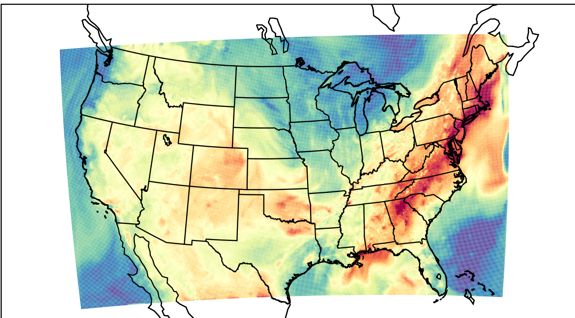
WRF (2019-07-30_18:00:00)
