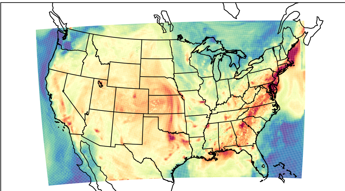
WRF (2019-07-31_21:00:00)
