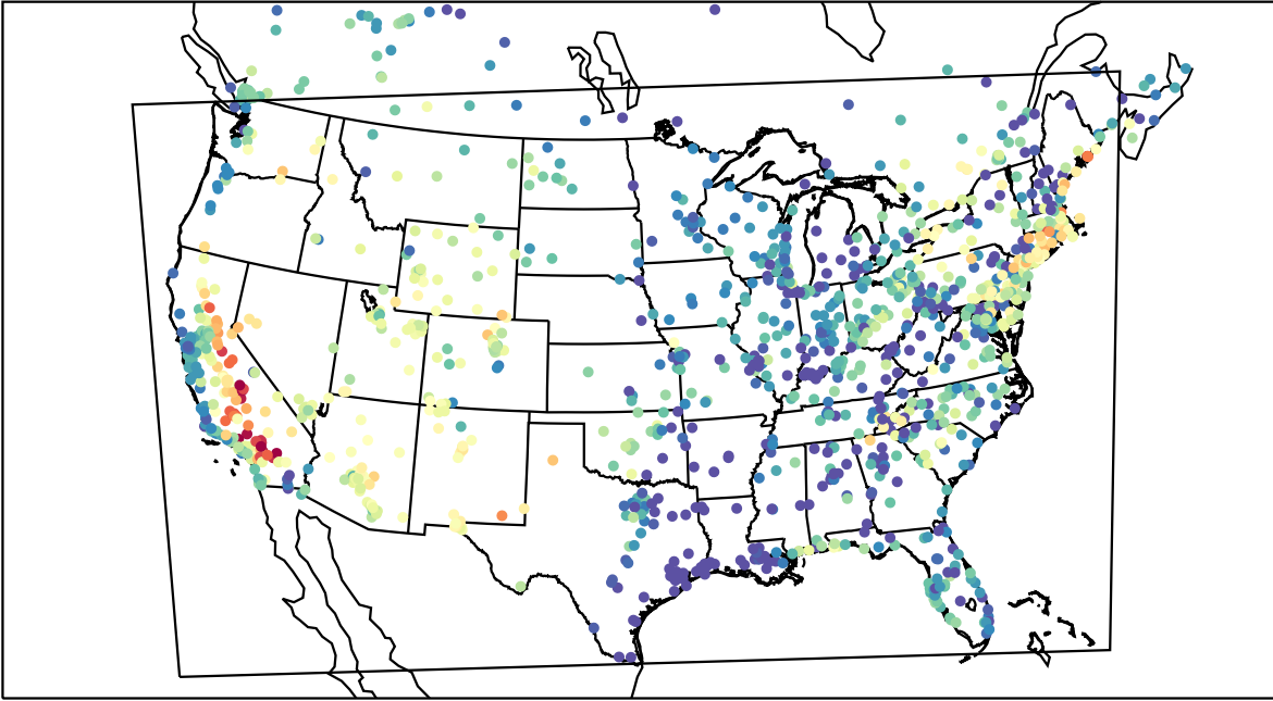
AirNOW (2019-07-30_02:00:00)
