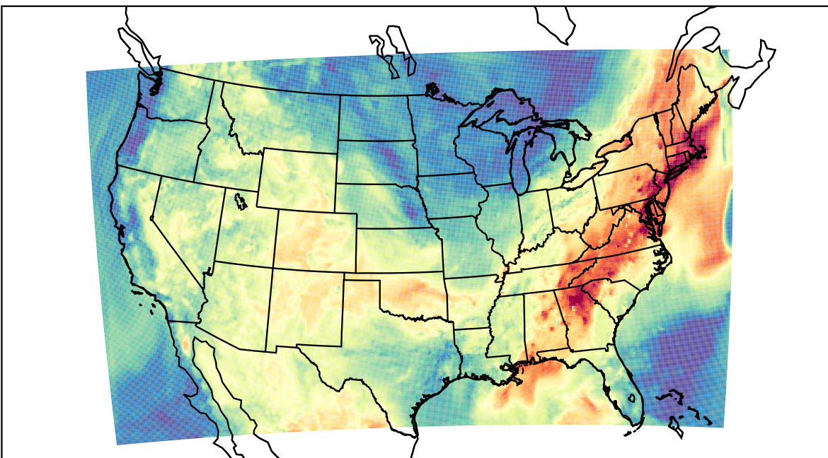
WRF (2019-07-30_16:00:00)
