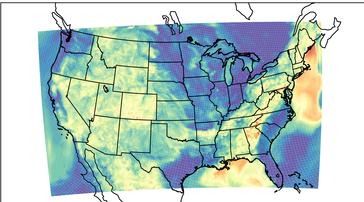
WRF (2019-07-31_07:00:00)
