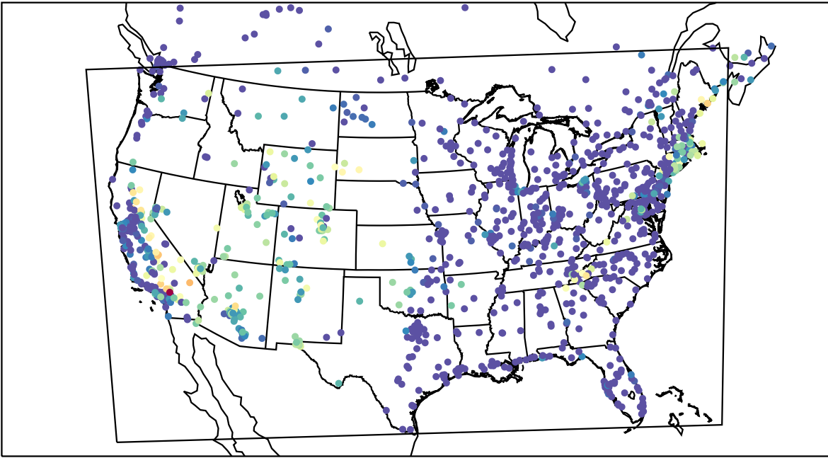
AirNOW (2019-07-31_10:00:00)
