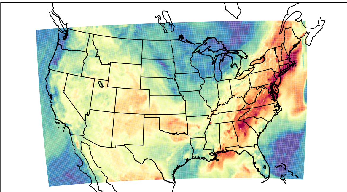
WRF (2019-07-30_17:00:00)
