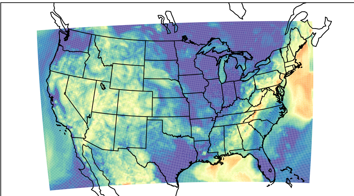
WRF (2019-07-31_13:00:00)
