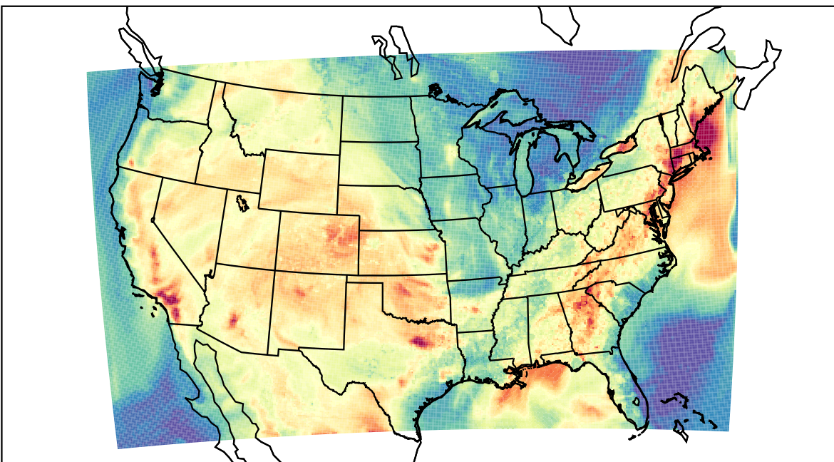
WRF (2019-07-31_00:00:00)
