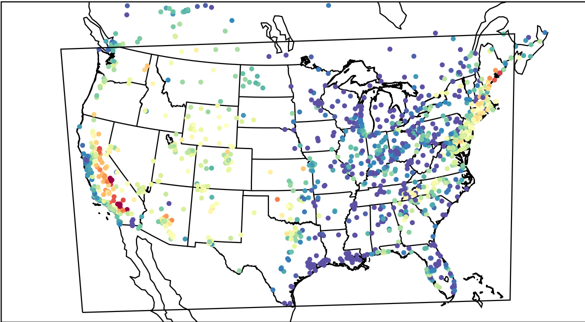
AirNOW (2019-07-31_02:00:00)
