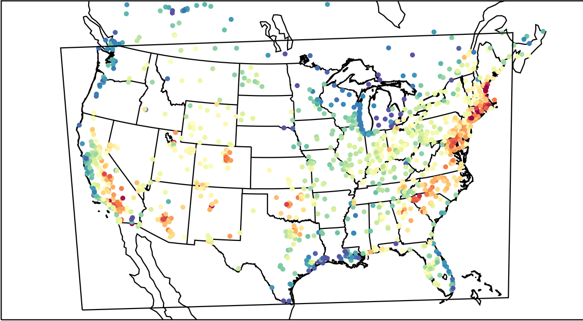
AirNOW (2019-07-30_19:00:00)
