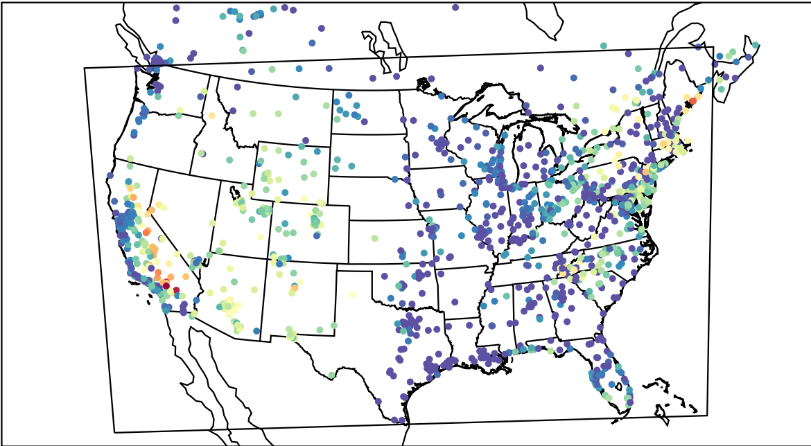
AirNOW (2019-07-30_05:00:00)
