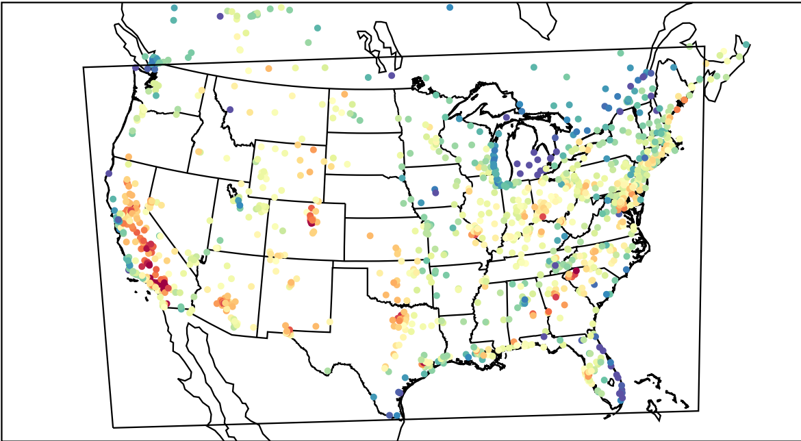
AirNOW (2019-07-31_21:00:00)
