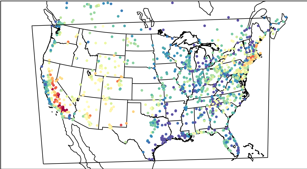
AirNOW (2019-07-30_01:00:00)
