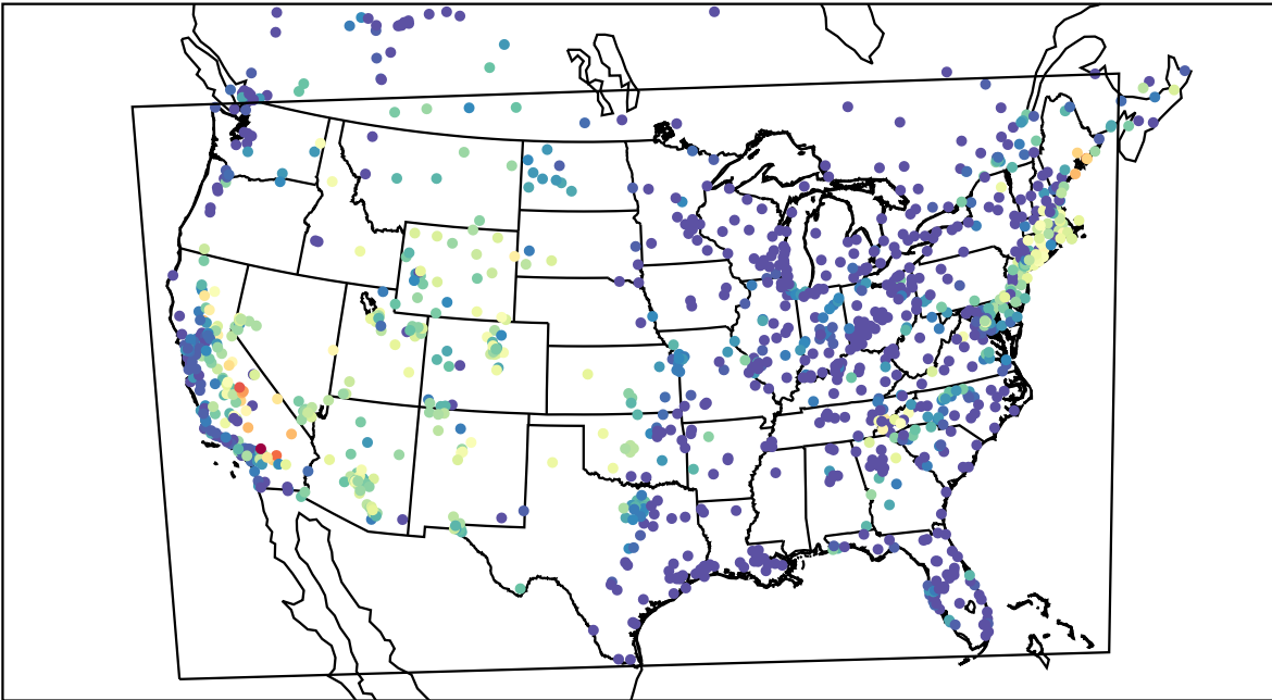
AirNOW (2019-07-31_06:00:00)
