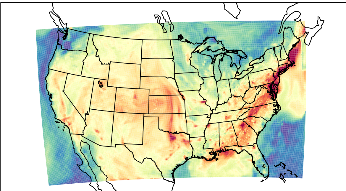
WRF (2019-07-31_20:00:00)
