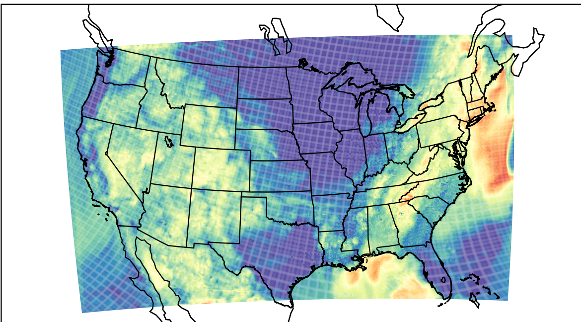
WRF (2019-07-30_13:00:00)
