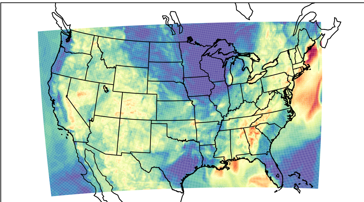
WRF (2019-07-30_05:00:00)
