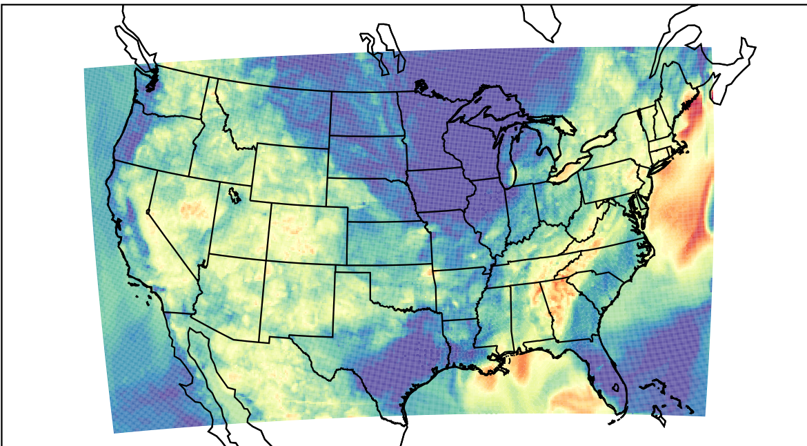
WRF (2019-07-30_07:00:00)
