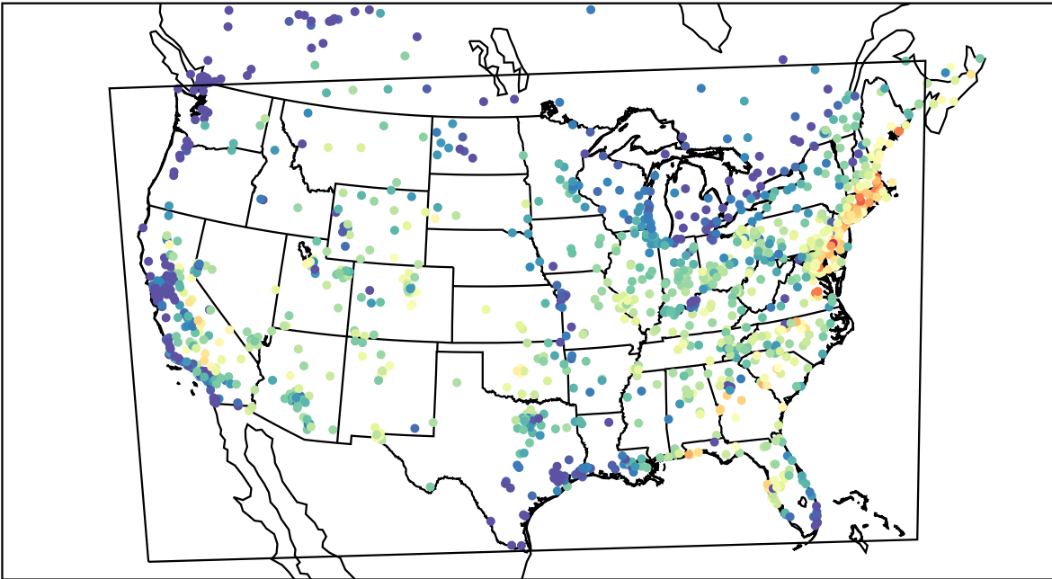
AirNOW (2019-07-31_15:00:00)
