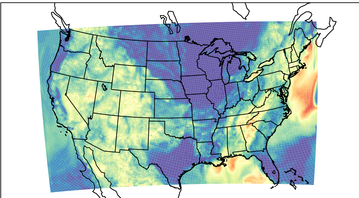
WRF (2019-07-30_10:00:00)
