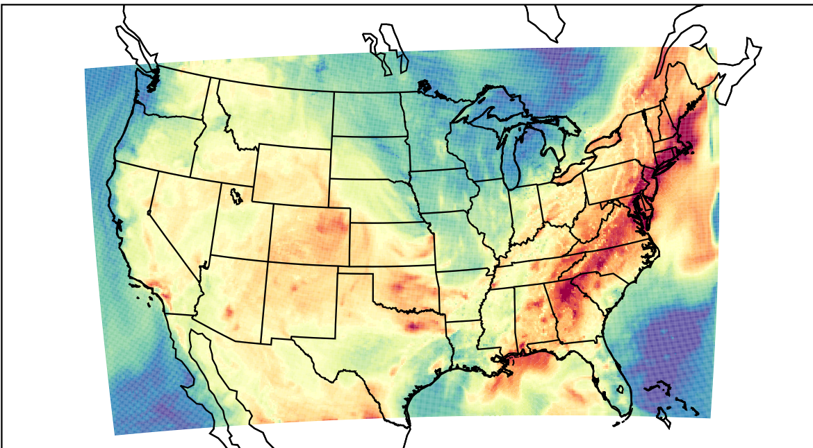
WRF (2019-07-30_19:00:00)
