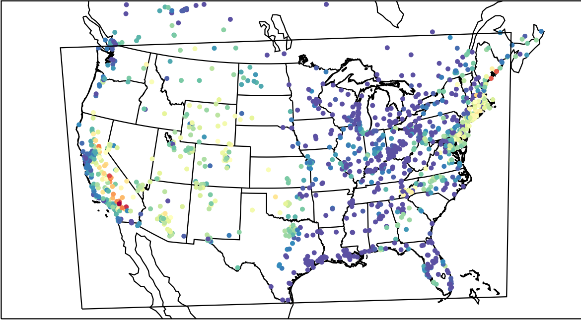
AirNOW (2019-07-31_04:00:00)
