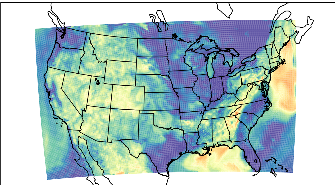
WRF (2019-07-31_10:00:00)
