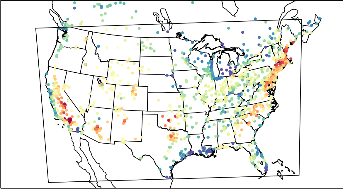
AirNOW (2019-07-30_22:00:00)
