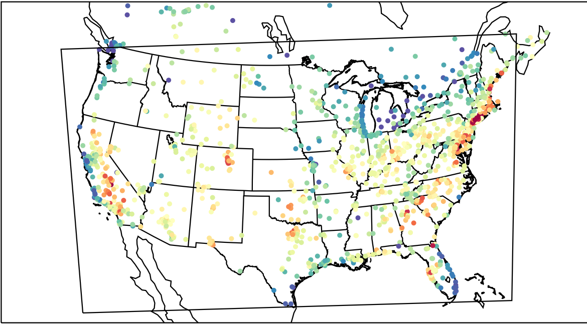
AirNOW (2019-07-31_18:00:00)
