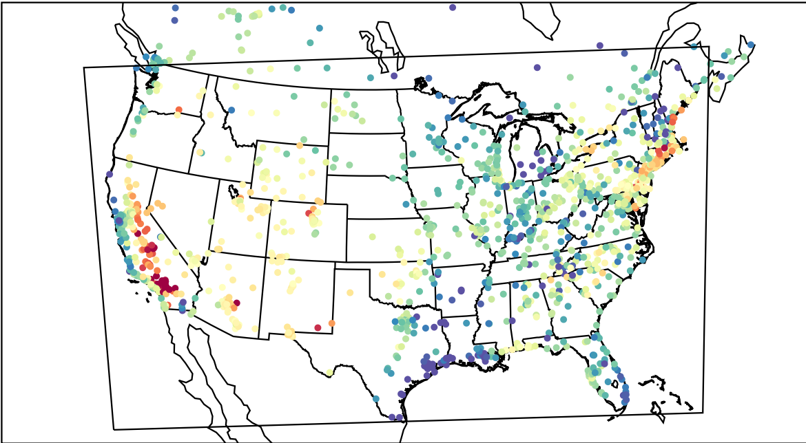
AirNOW (2019-07-30_00:00:00)
