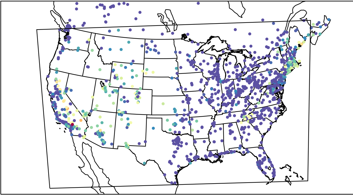
AirNOW (2019-07-31_11:00:00)
