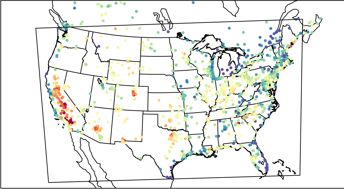
AirNOW (2019-07-31_23:00:00)
