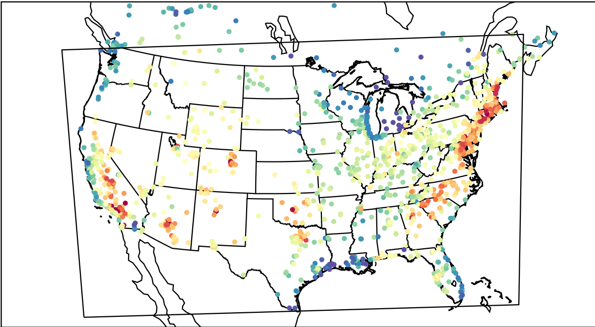
AirNOW (2019-07-30_20:00:00)
