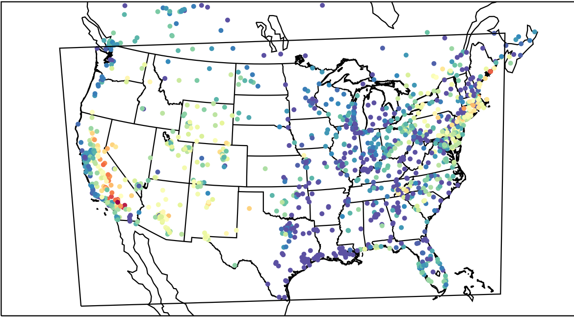
AirNOW (2019-07-30_03:00:00)
