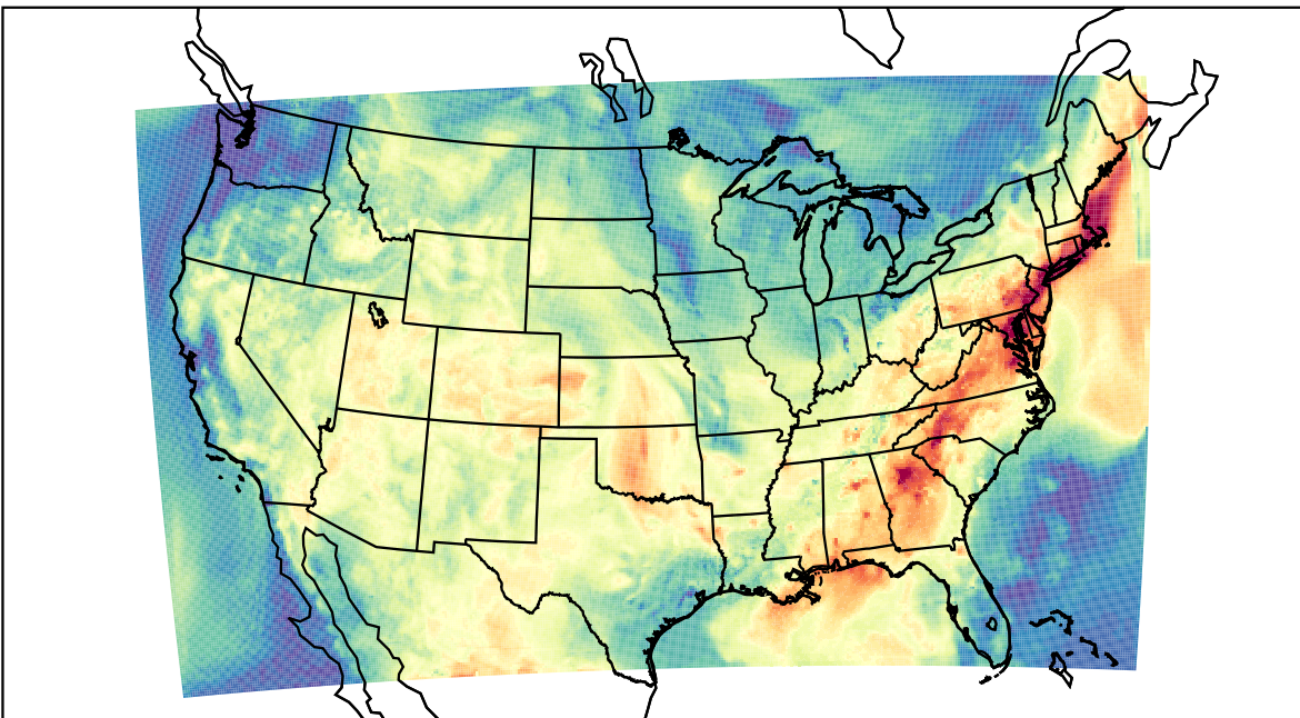
WRF (2019-07-31_16:00:00)
