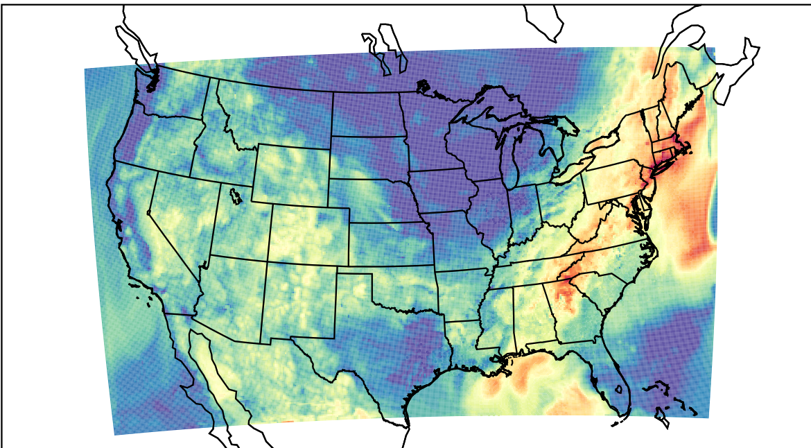
WRF (2019-07-30_14:00:00)
