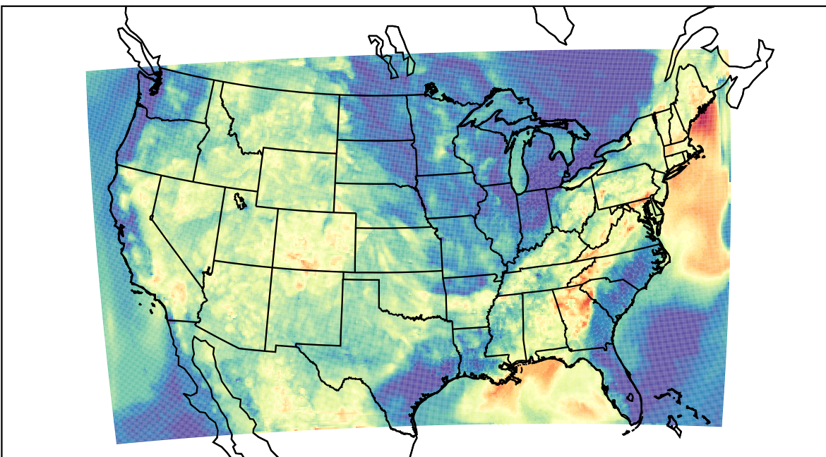
WRF (2019-07-31_05:00:00)
