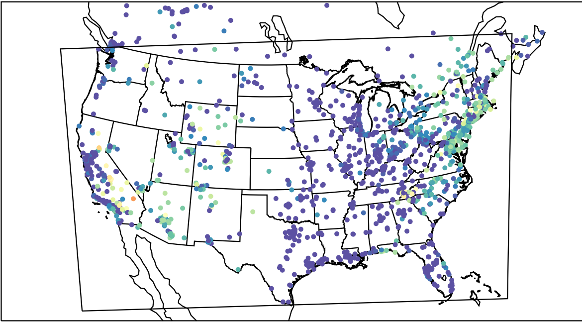
AirNOW (2019-07-30_12:00:00)
