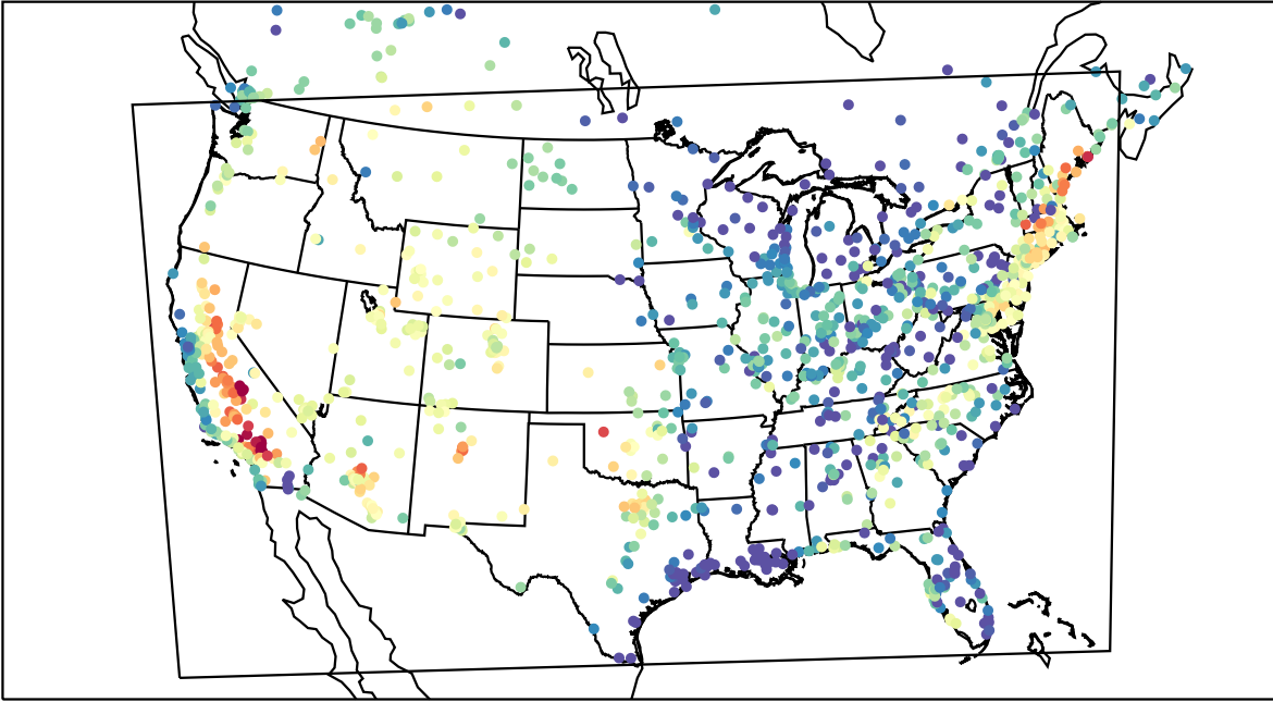
AirNOW (2019-07-31_01:00:00)
