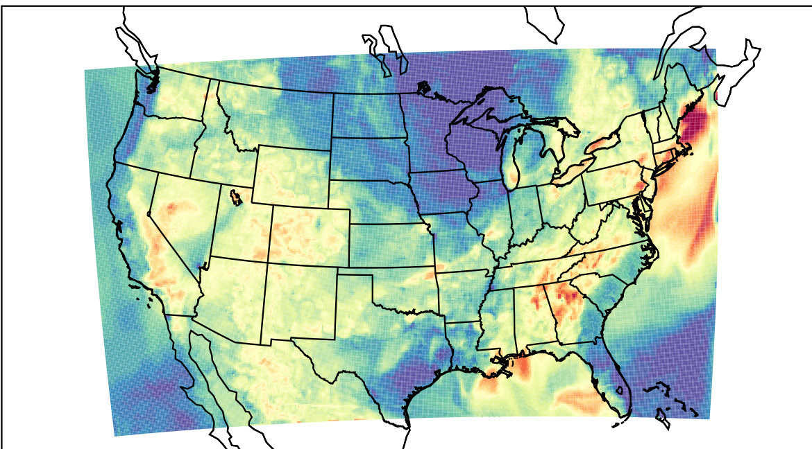
WRF (2019-07-30_03:00:00)
