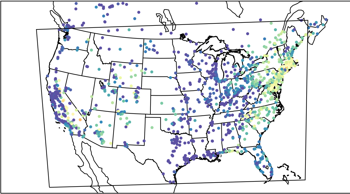
AirNOW (2019-07-30_13:00:00)
