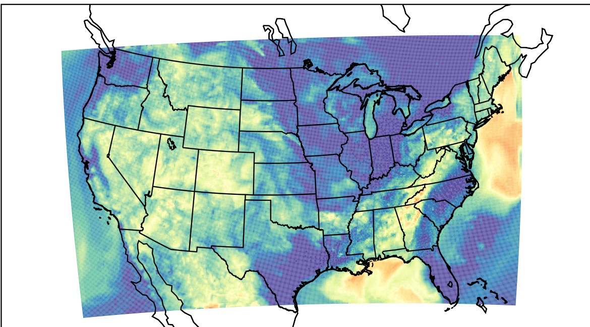
WRF (2019-07-31_11:00:00)
