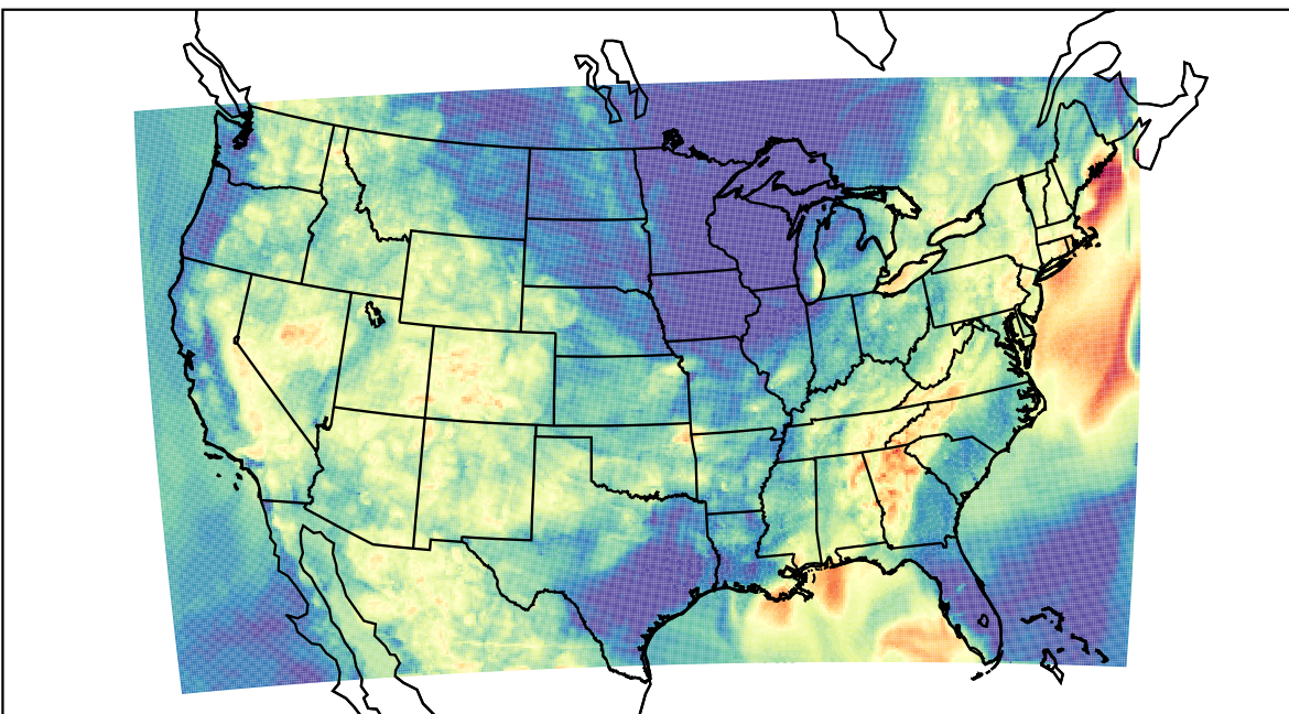
WRF (2019-07-30_06:00:00)
