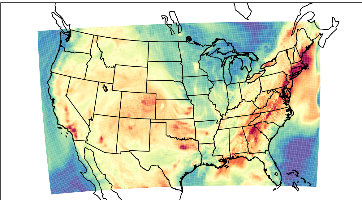
WRF (2019-07-30_22:00:00)
