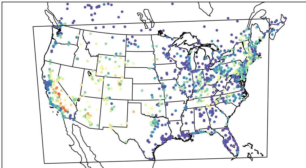
AirNOW (2019-08-07_04:00:00)
