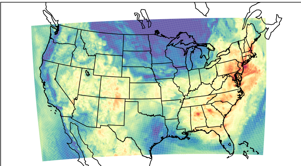
WRF (2019-08-08_15:00:00)
