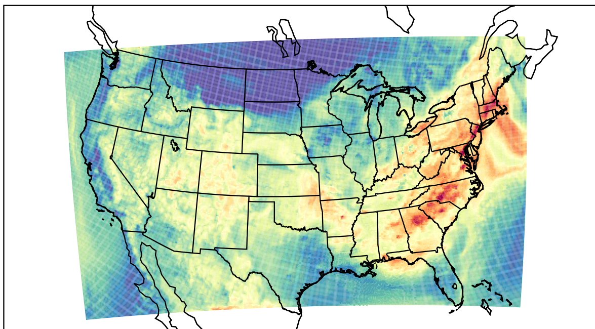
WRF (2019-08-07_15:00:00)
