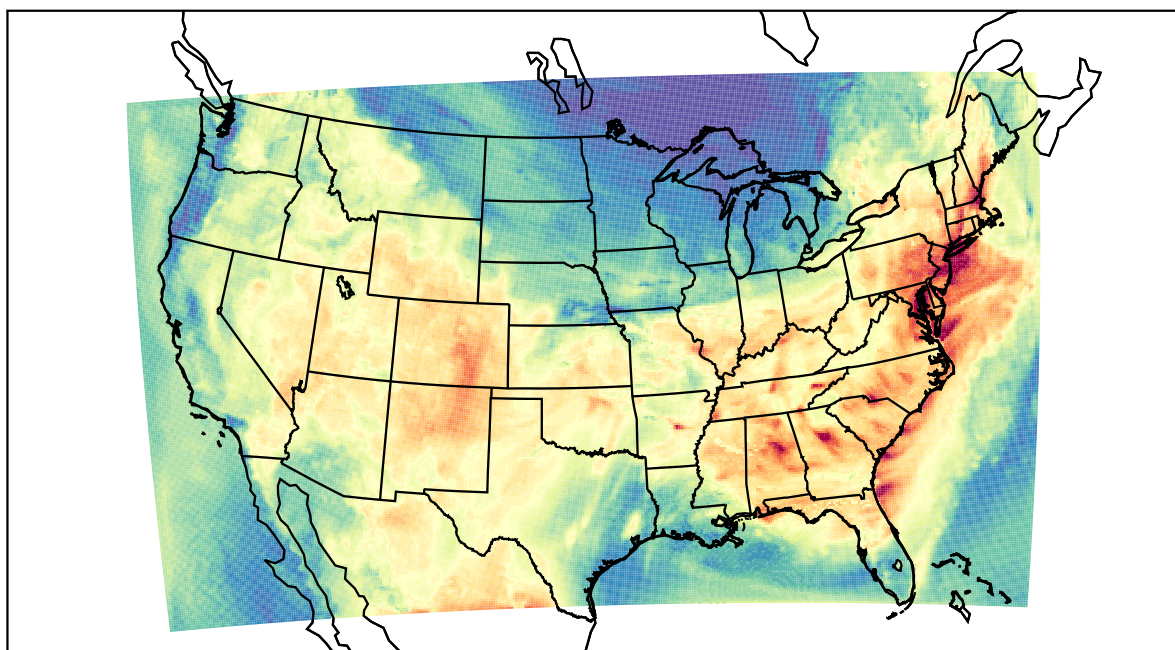
WRF (2019-08-08_17:00:00)
