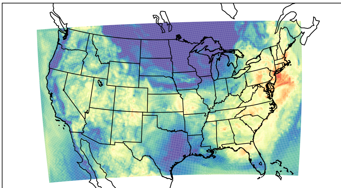
WRF (2019-08-08_14:00:00)
