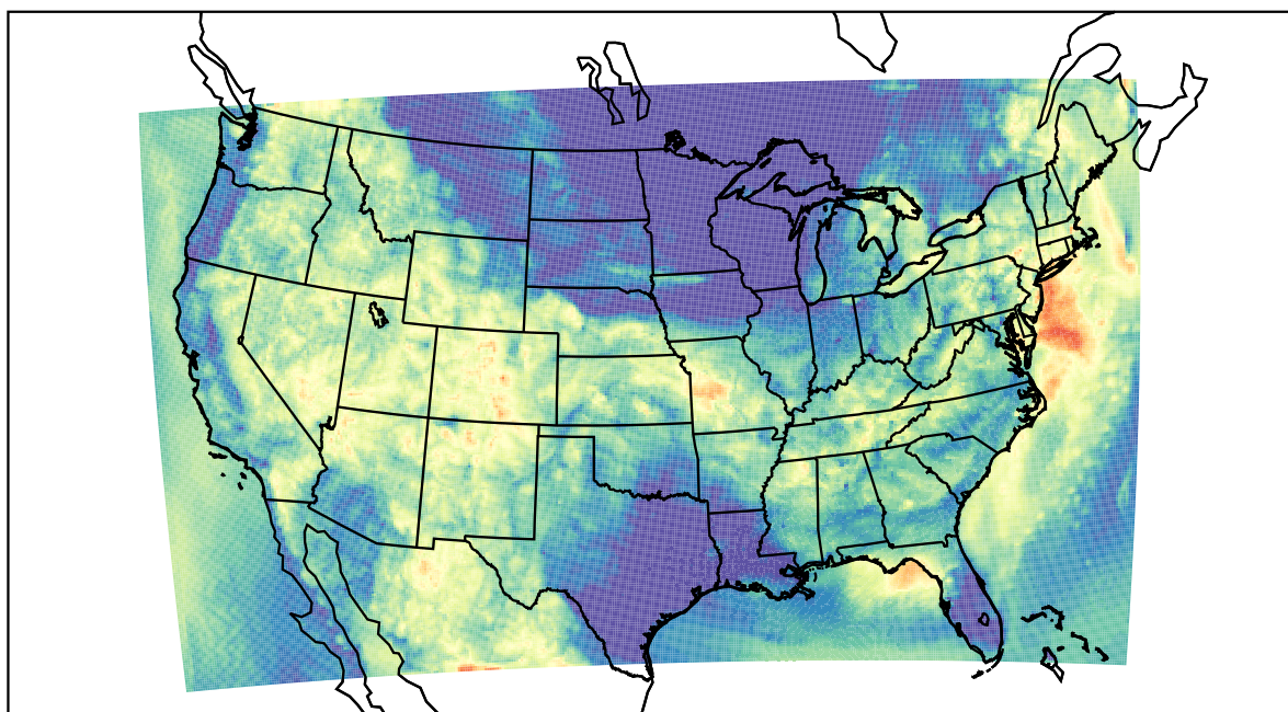
WRF (2019-08-08_10:00:00)
