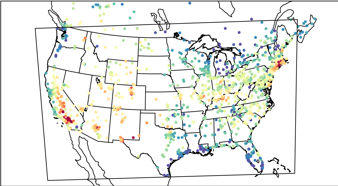
AirNOW (2019-08-08_23:00:00)
