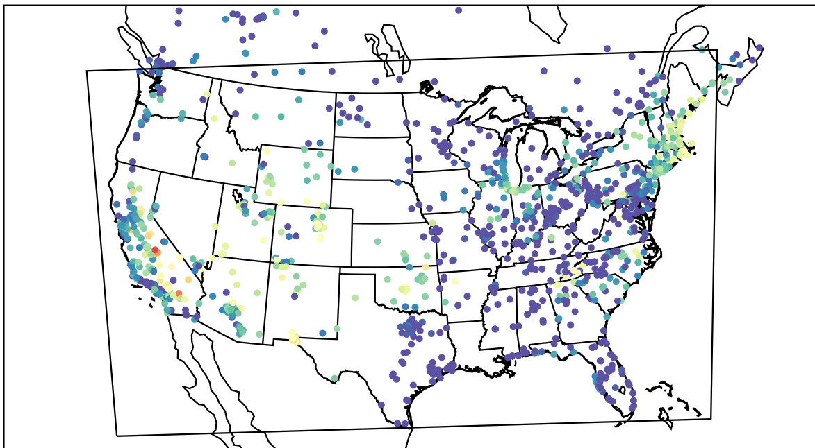
AirNOW (2019-08-08_07:00:00)
