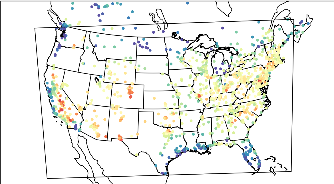
AirNOW (2019-08-07_18:00:00)
