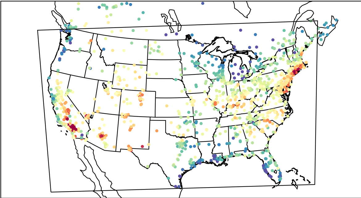
AirNOW (2019-08-08_21:00:00)
