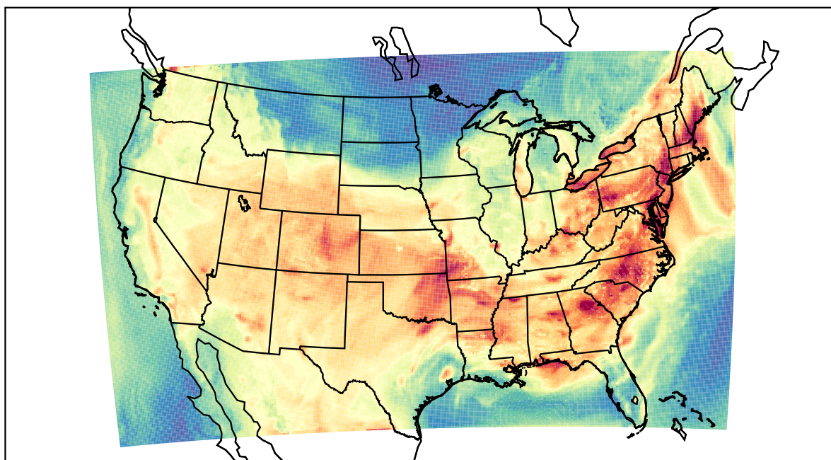
WRF (2019-08-07_19:00:00)
