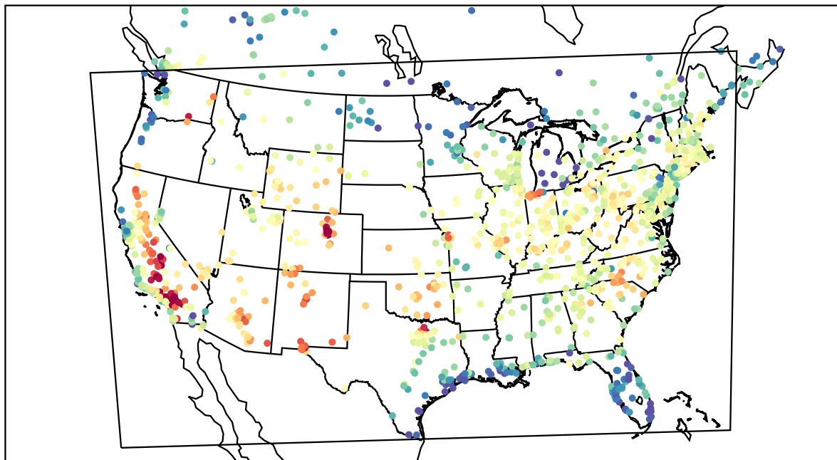
AirNOW (2019-08-07_21:00:00)
