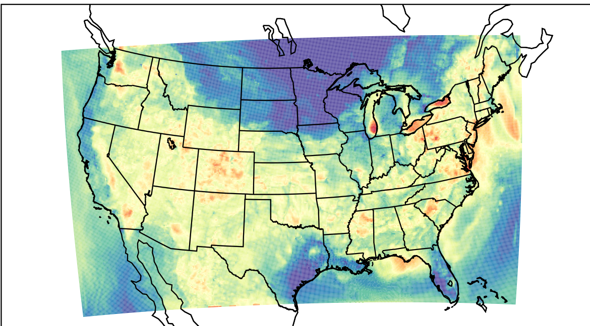
WRF (2019-08-08_03:00:00)
