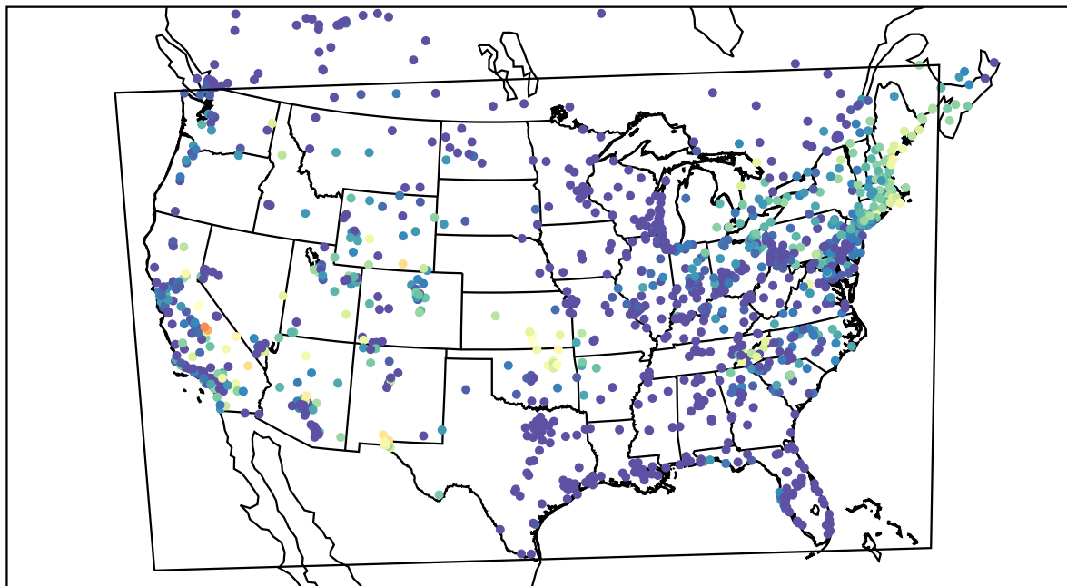
AirNOW (2019-08-08_12:00:00)
