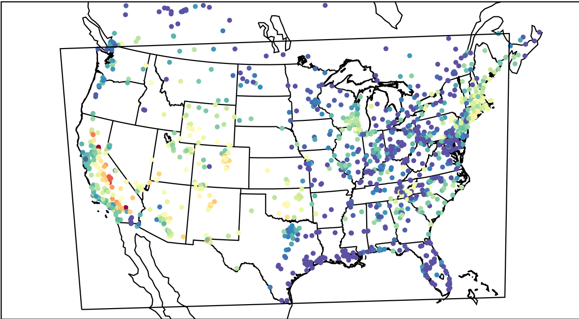
AirNOW (2019-08-08_03:00:00)
