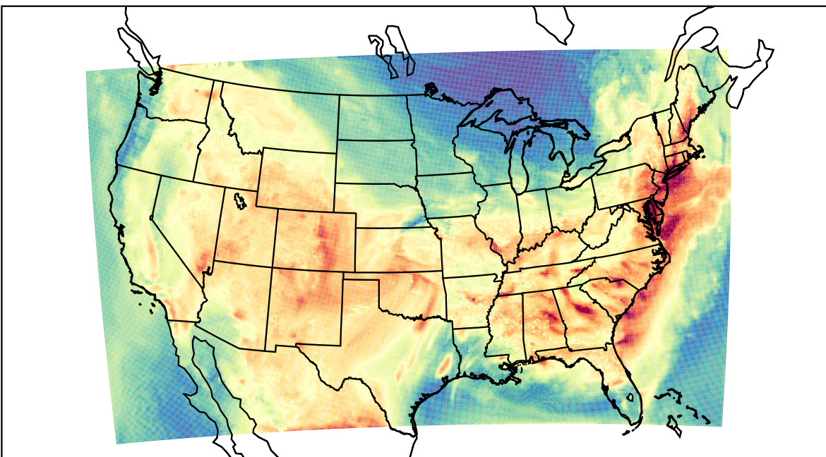
WRF (2019-08-08_20:00:00)
