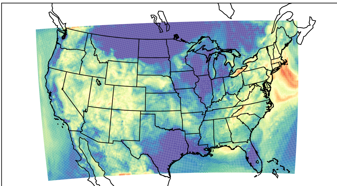
WRF (2019-08-07_13:00:00)
