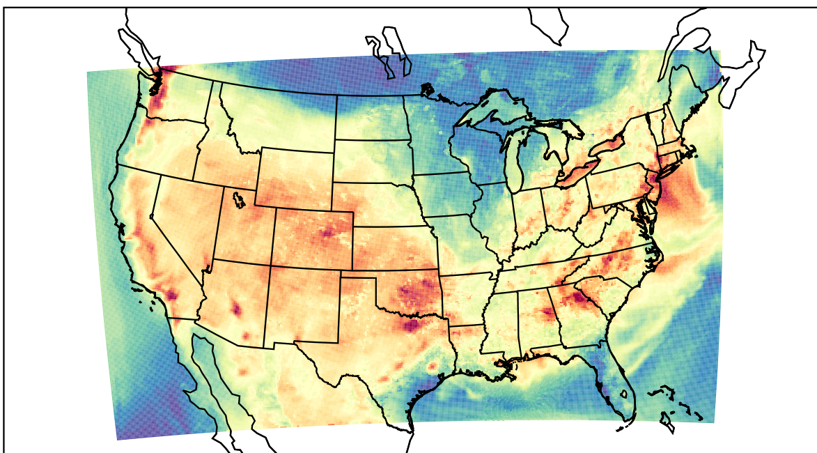
WRF (2019-08-07_00:00:00)
