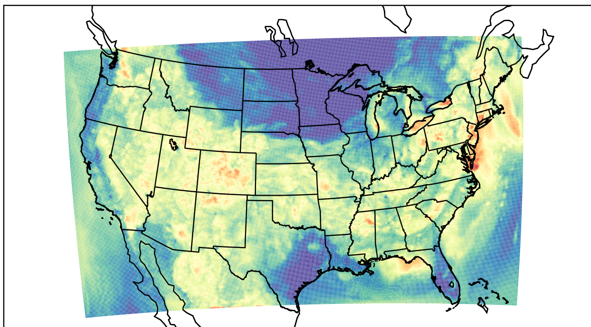
WRF (2019-08-08_05:00:00)
