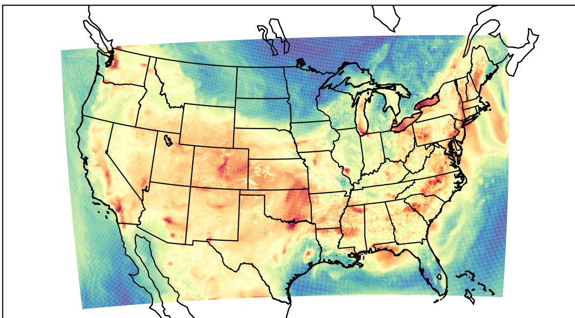
WRF (2019-08-07_23:00:00)
