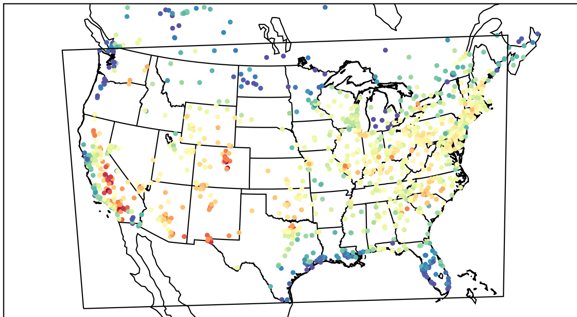
AirNOW (2019-08-07_19:00:00)
