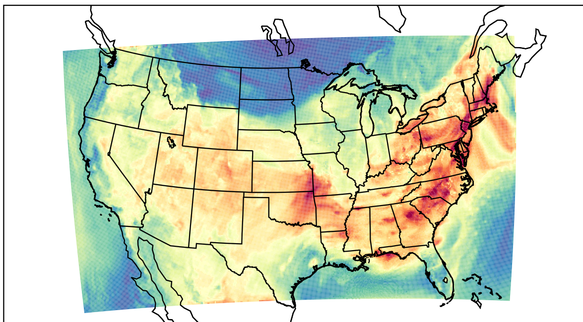
WRF (2019-08-07_17:00:00)
