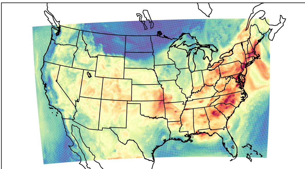
WRF (2019-08-07_16:00:00)
