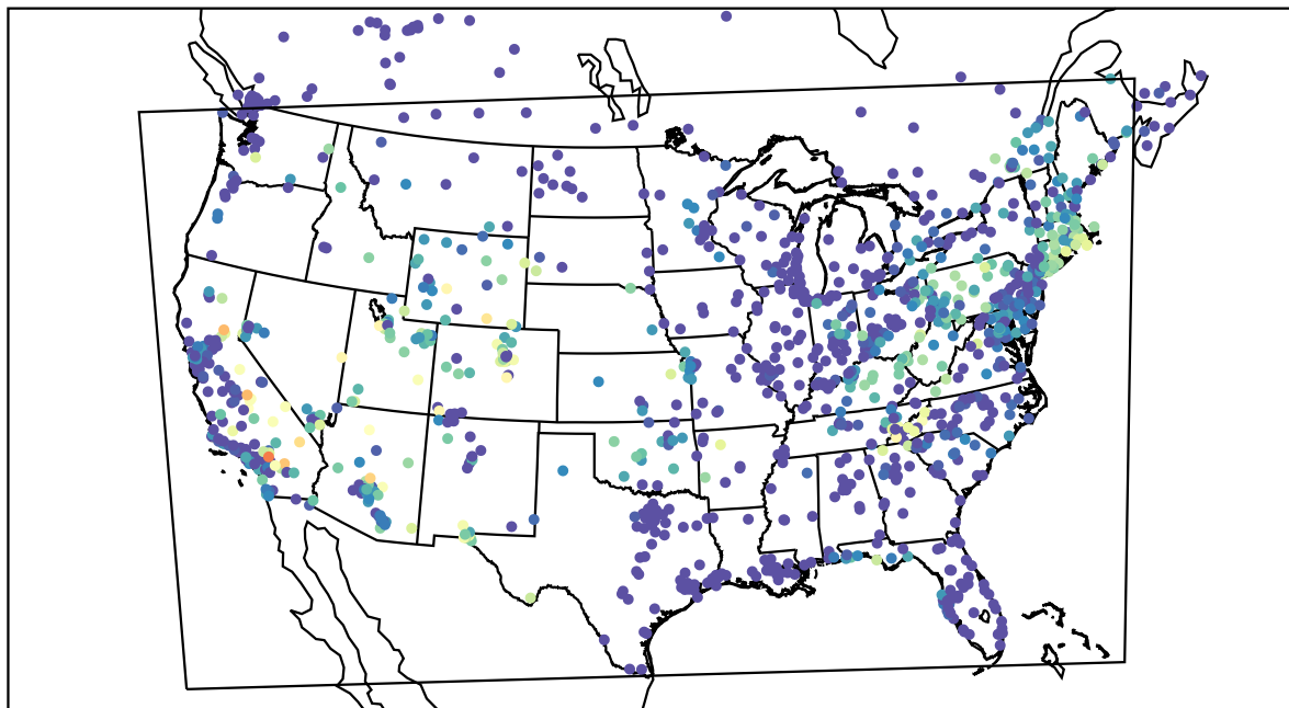
AirNOW (2019-08-07_12:00:00)
