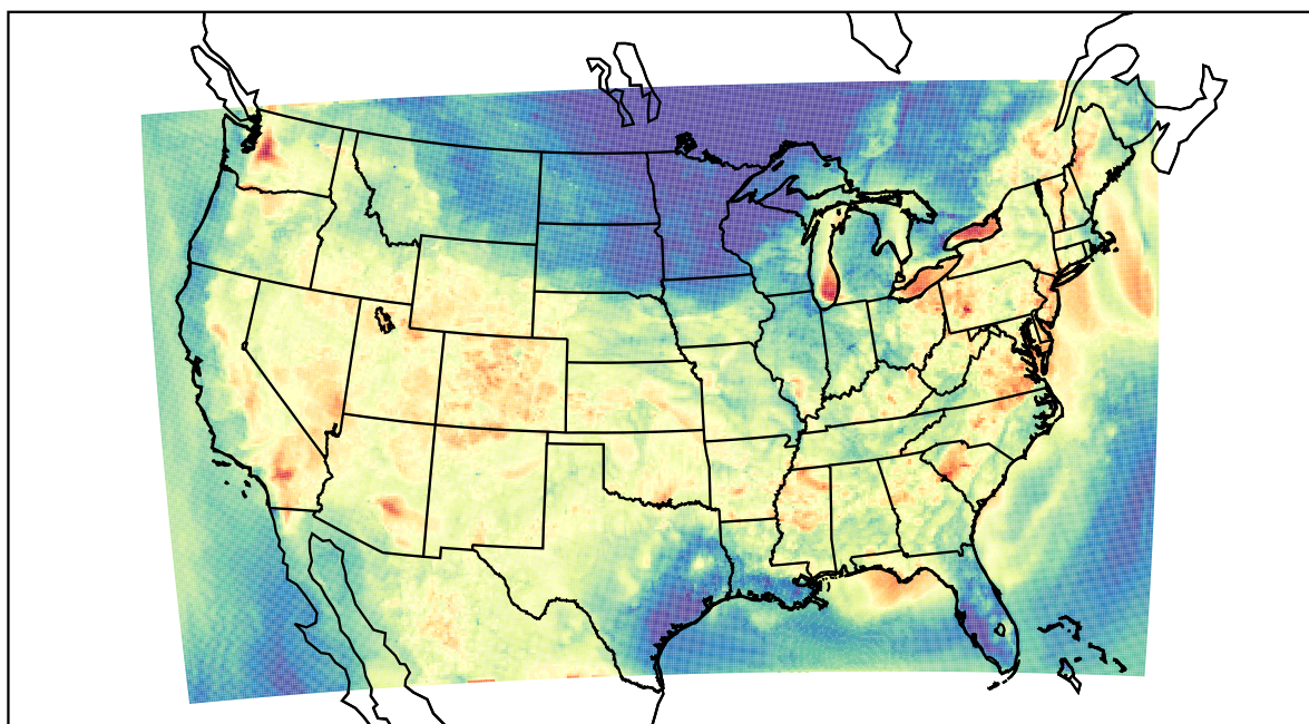
WRF (2019-08-08_02:00:00)
