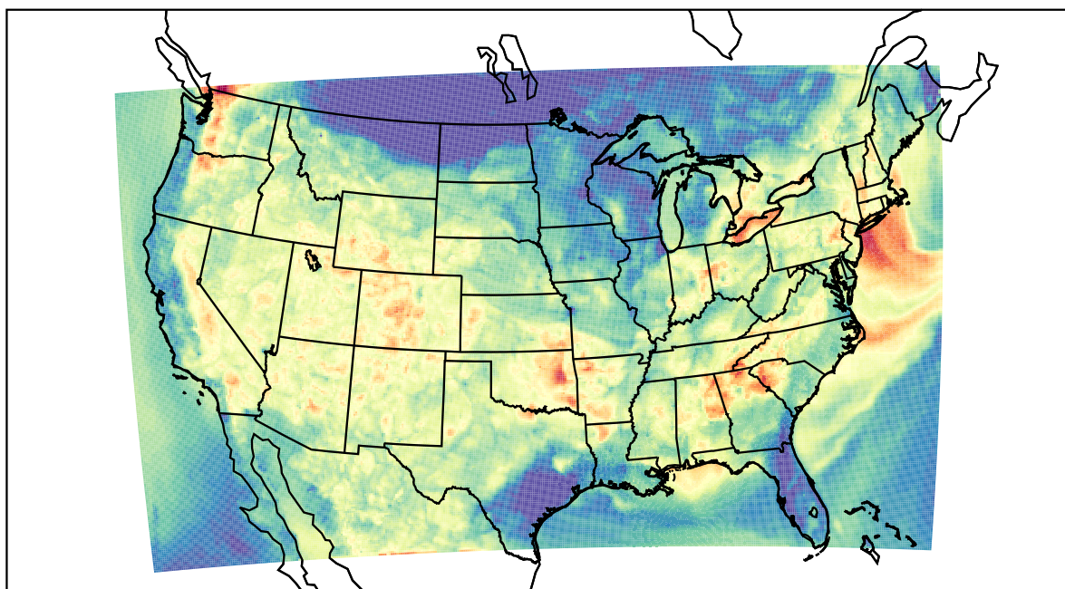
WRF (2019-08-07_04:00:00)
