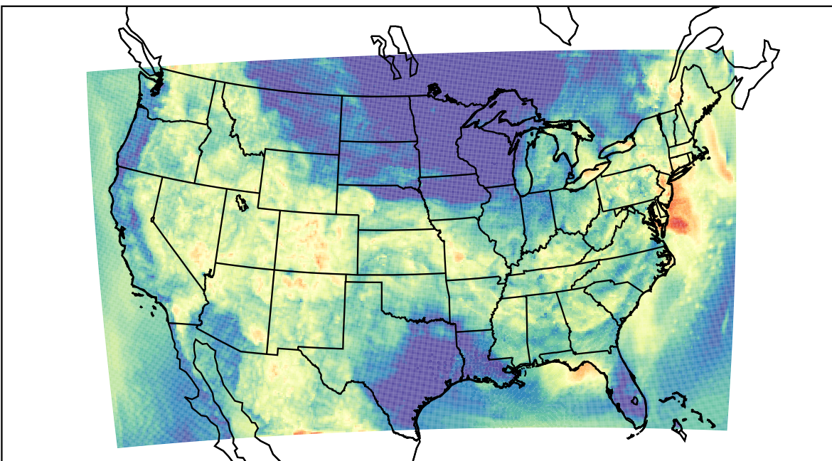
WRF (2019-08-08_08:00:00)
