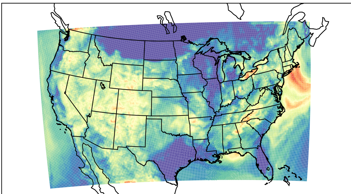
WRF (2019-08-07_10:00:00)
