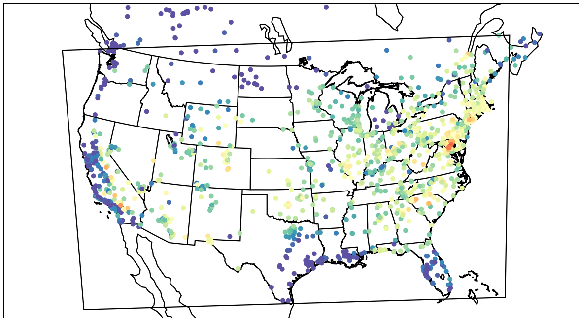
AirNOW (2019-08-07_15:00:00)
