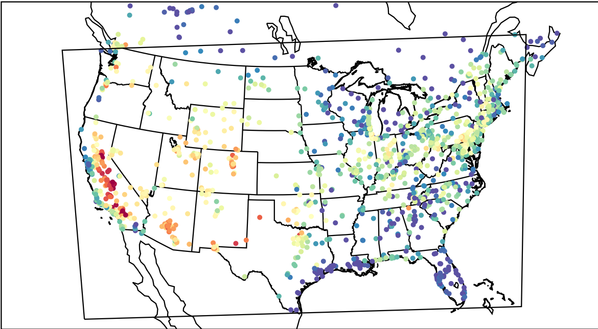
AirNOW (2019-08-07_01:00:00)
