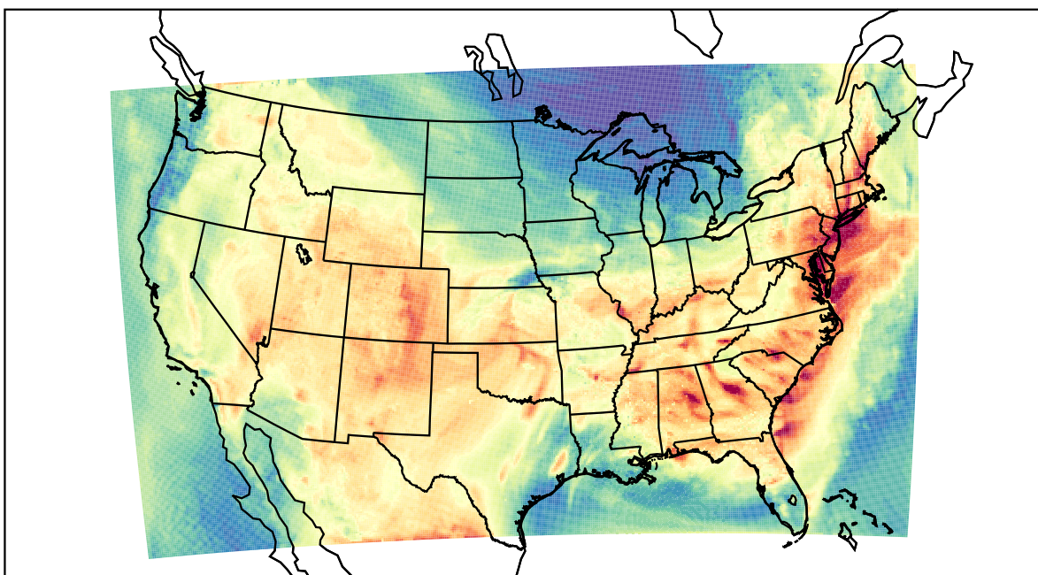
WRF (2019-08-08_19:00:00)
