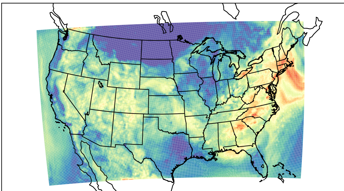
WRF (2019-08-07_14:00:00)
