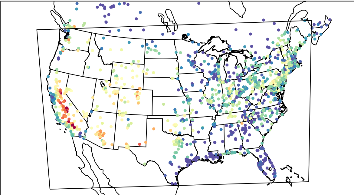
AirNOW (2019-08-07_02:00:00)
