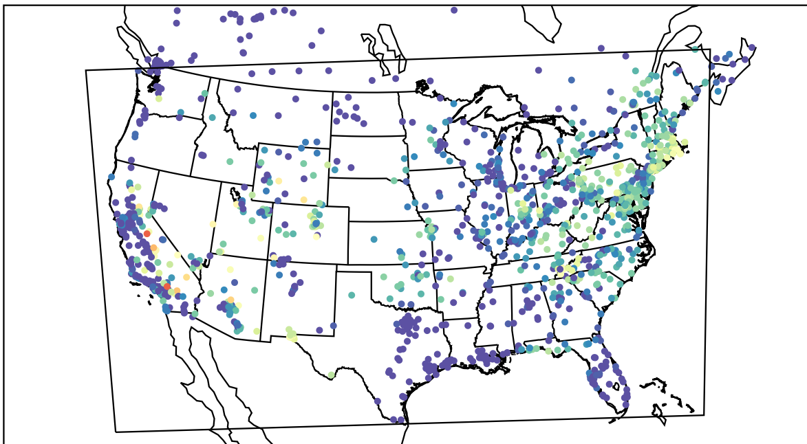
AirNOW (2019-08-07_13:00:00)
