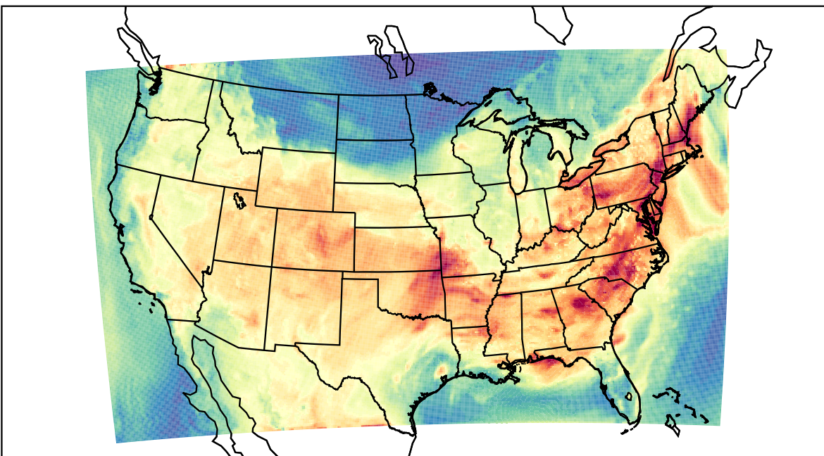
WRF (2019-08-07_18:00:00)
