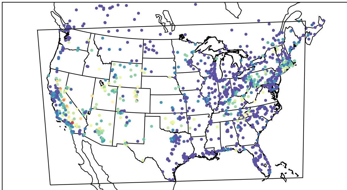
AirNOW (2019-08-07_09:00:00)
