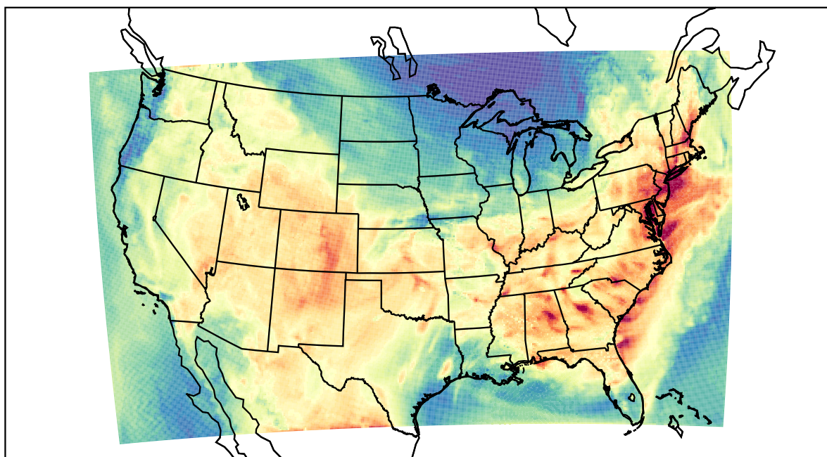
WRF (2019-08-08_18:00:00)
