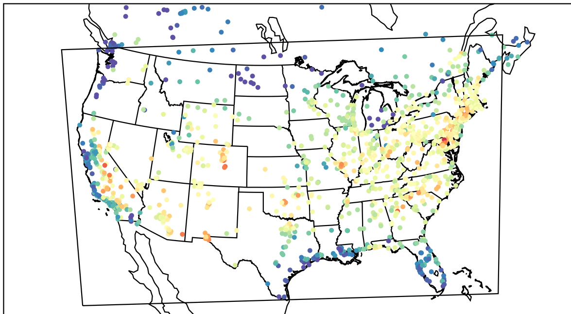
AirNOW (2019-08-07_17:00:00)
