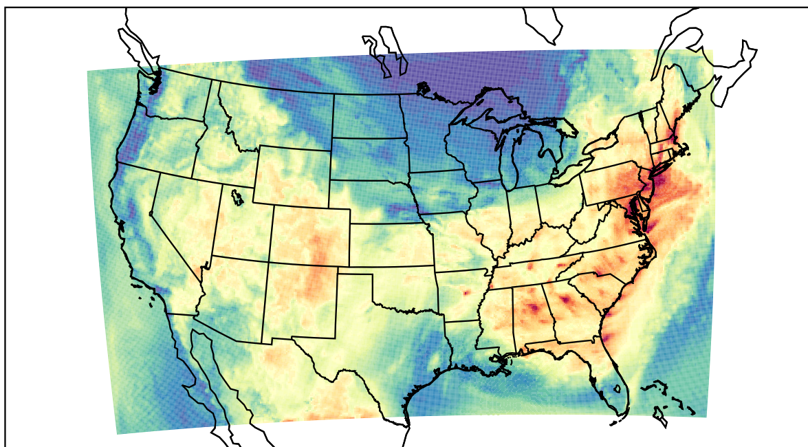
WRF (2019-08-08_16:00:00)
