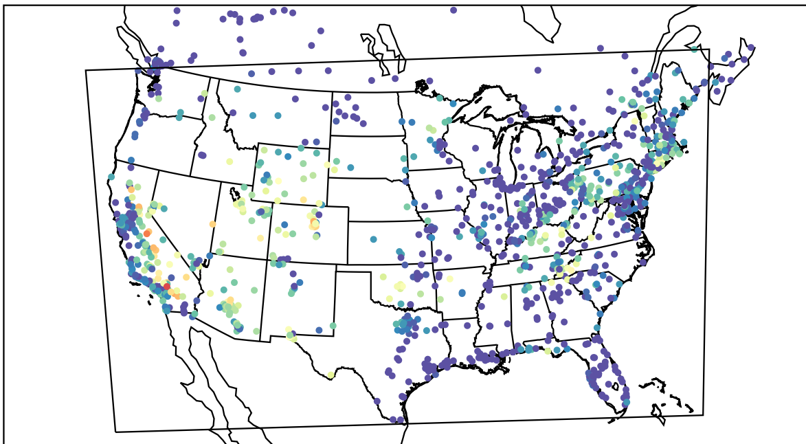
AirNOW (2019-08-07_08:00:00)
