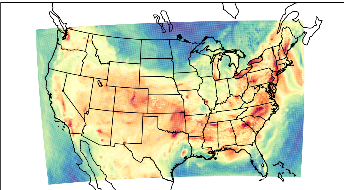
WRF (2019-08-07_22:00:00)
