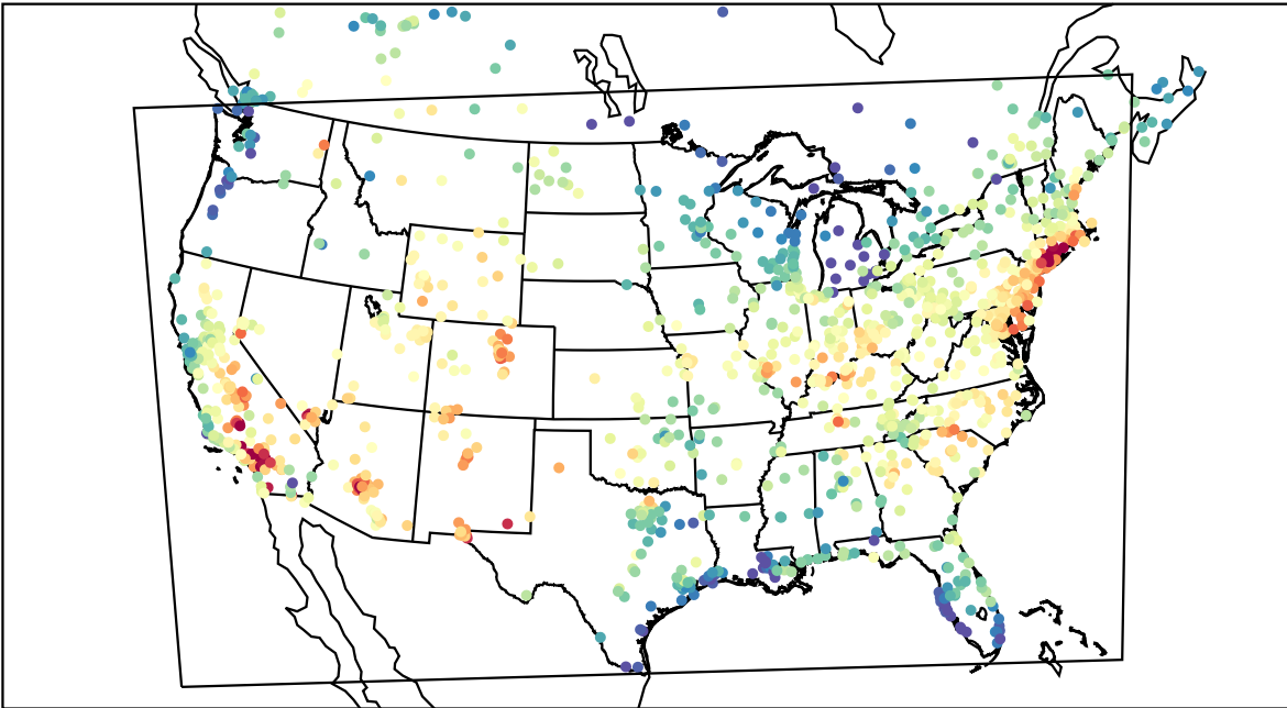
AirNOW (2019-08-08_20:00:00)
