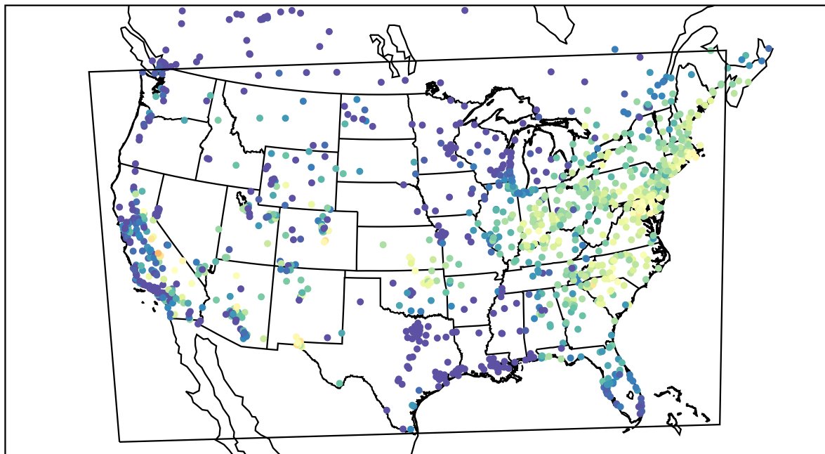
AirNOW (2019-08-08_14:00:00)
