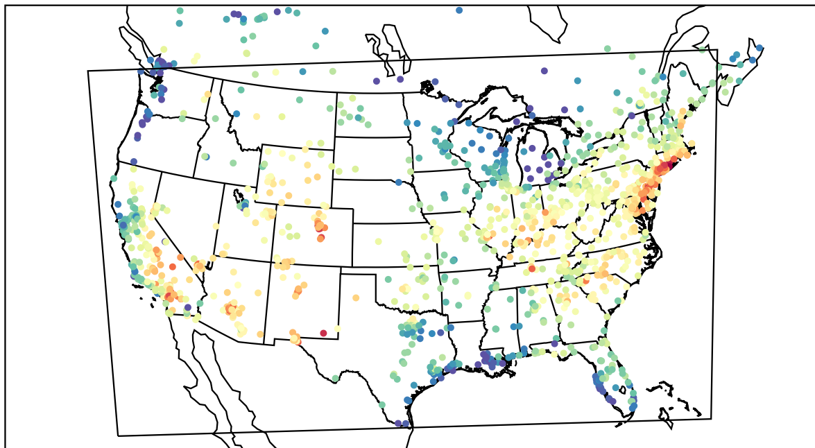
AirNOW (2019-08-08_18:00:00)
