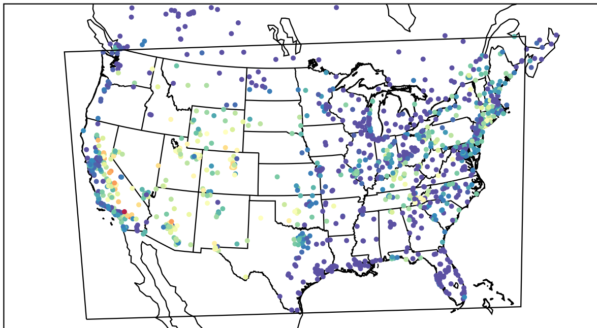
AirNOW (2019-08-07_06:00:00)
