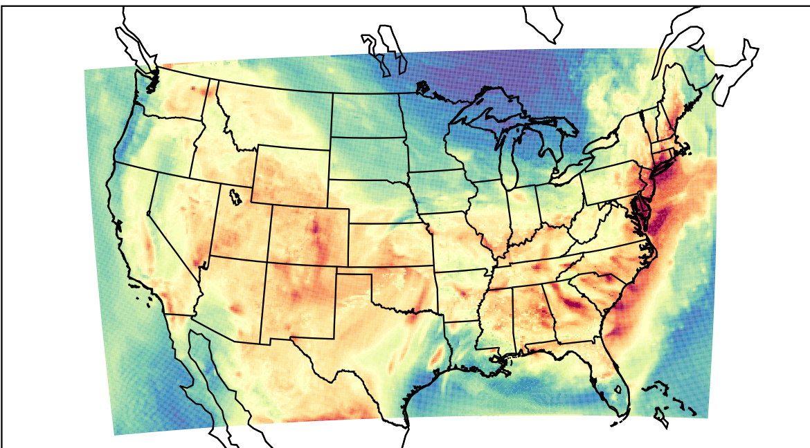
WRF (2019-08-08_21:00:00)
