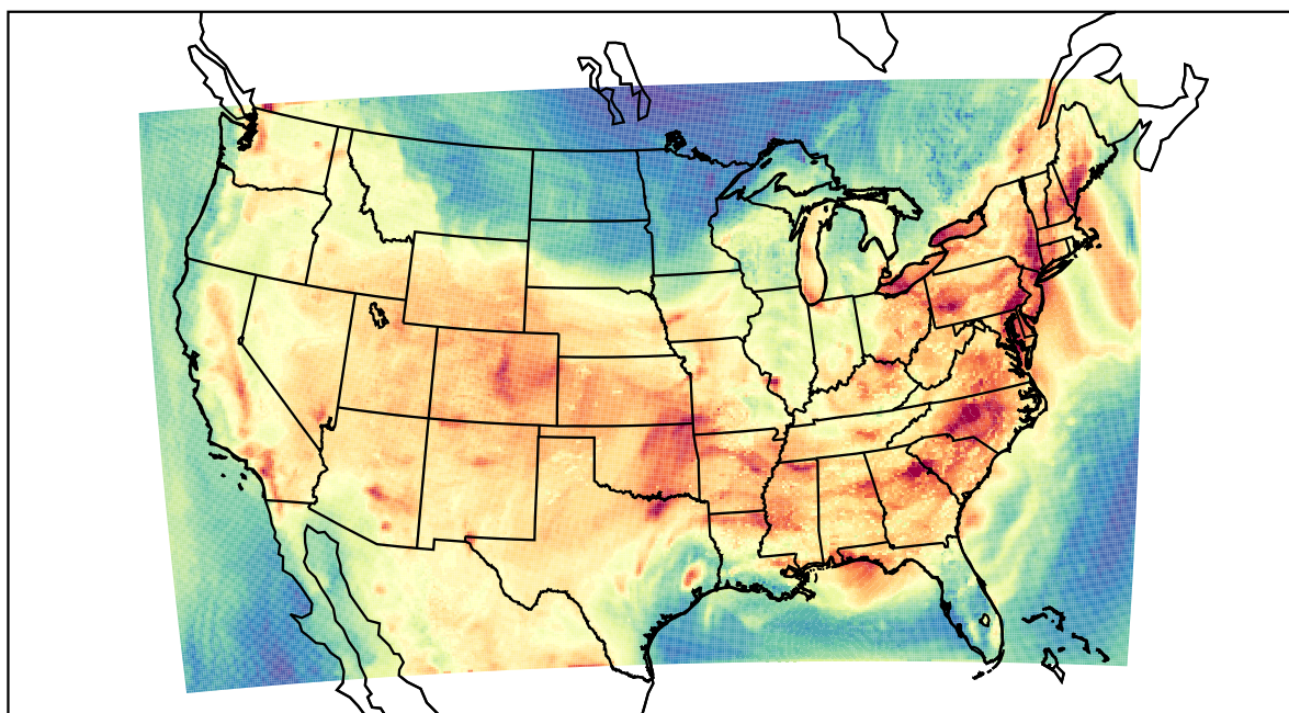
WRF (2019-08-07_21:00:00)
