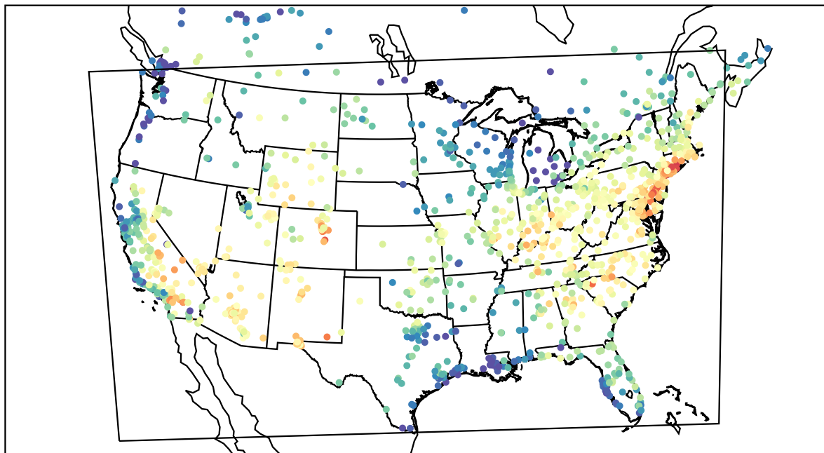
AirNOW (2019-08-08_17:00:00)
