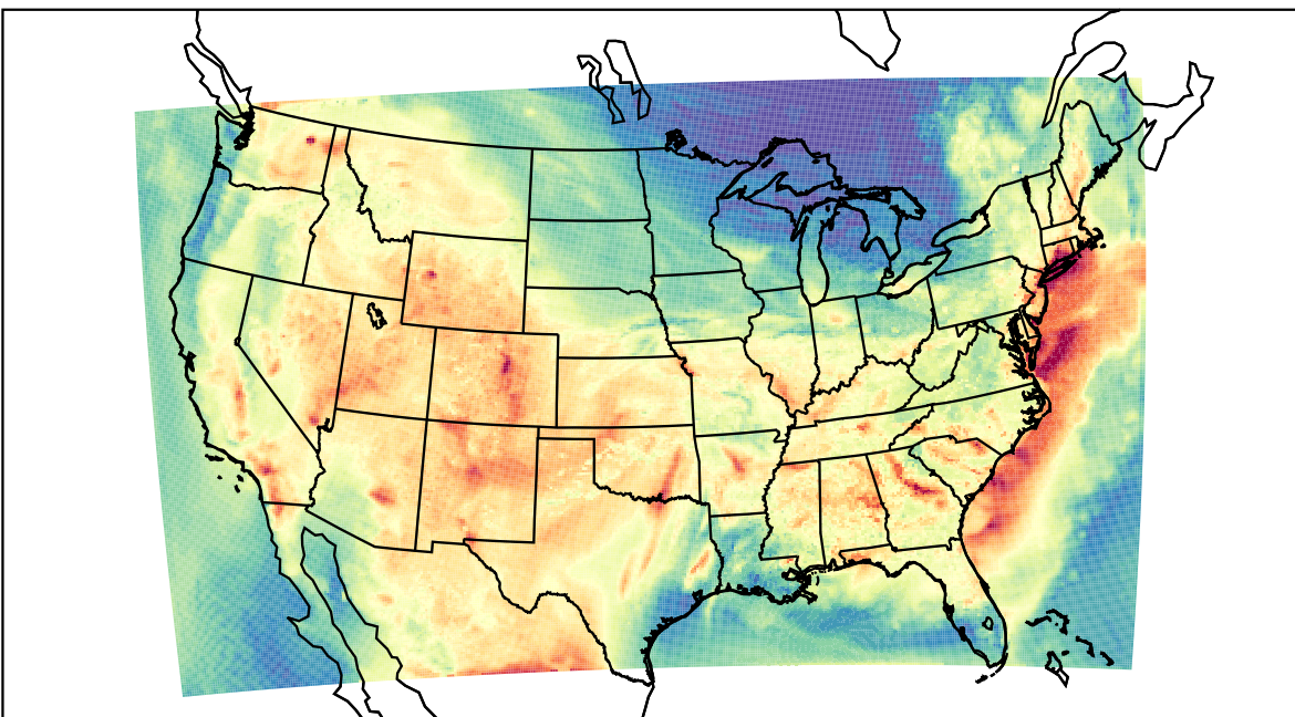
WRF (2019-08-08_23:00:00)
