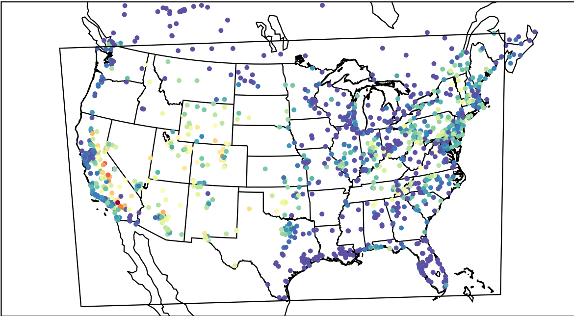
AirNOW (2019-08-07_05:00:00)
