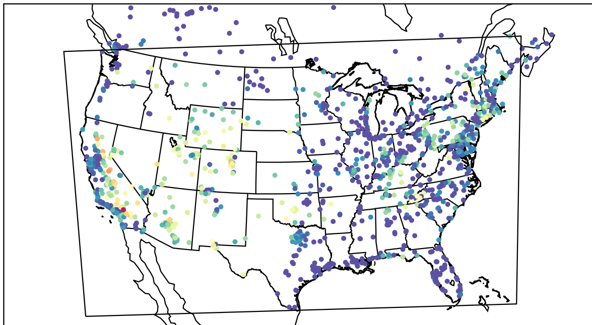
AirNOW (2019-08-07_07:00:00)
