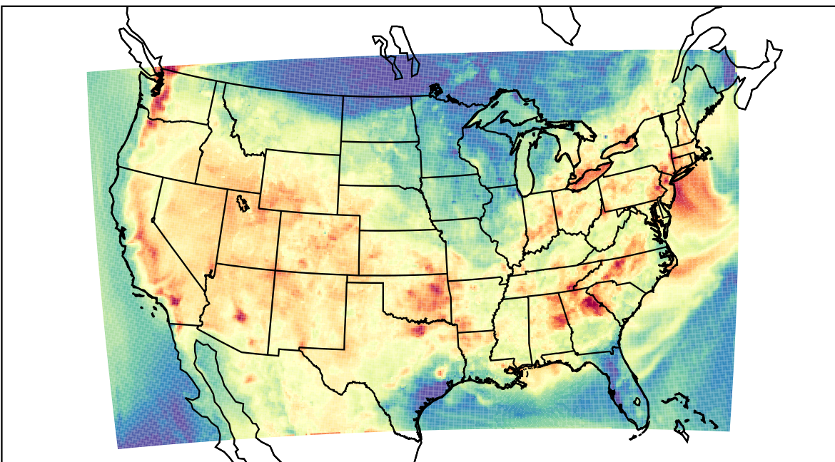
WRF (2019-08-07_01:00:00)
