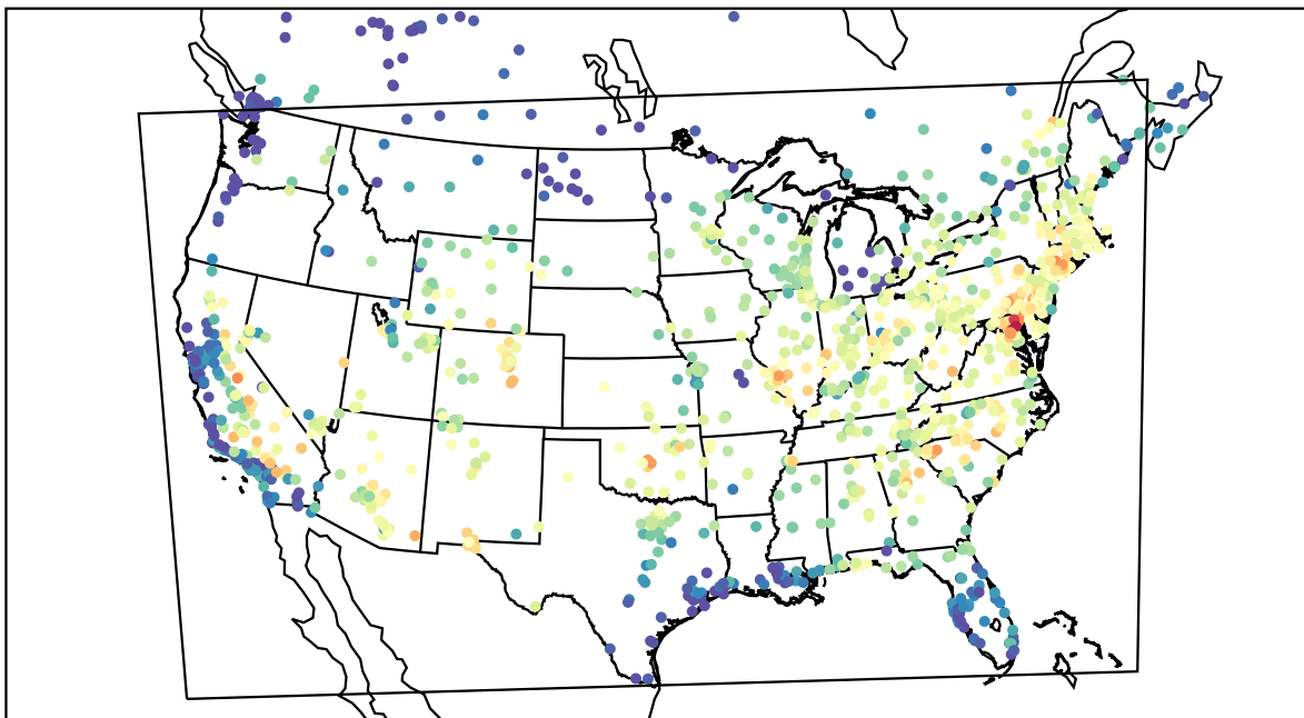
AirNOW (2019-08-07_16:00:00)
