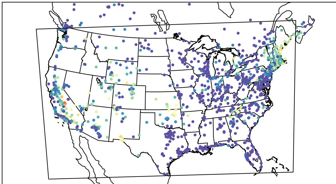
AirNOW (2019-08-08_10:00:00)
