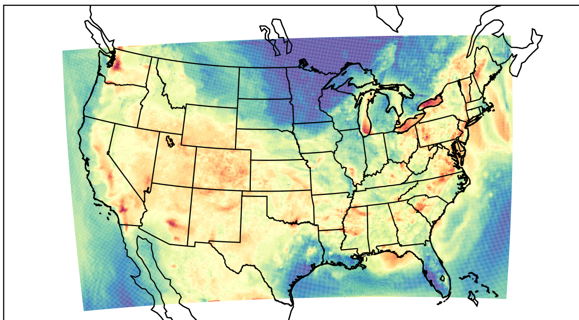
WRF (2019-08-08_01:00:00)
