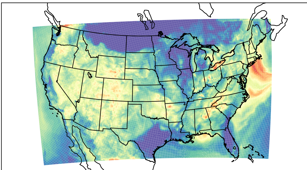
WRF (2019-08-07_08:00:00)
