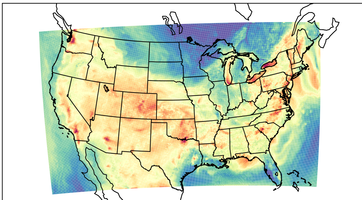
WRF (2019-08-08_00:00:00)
