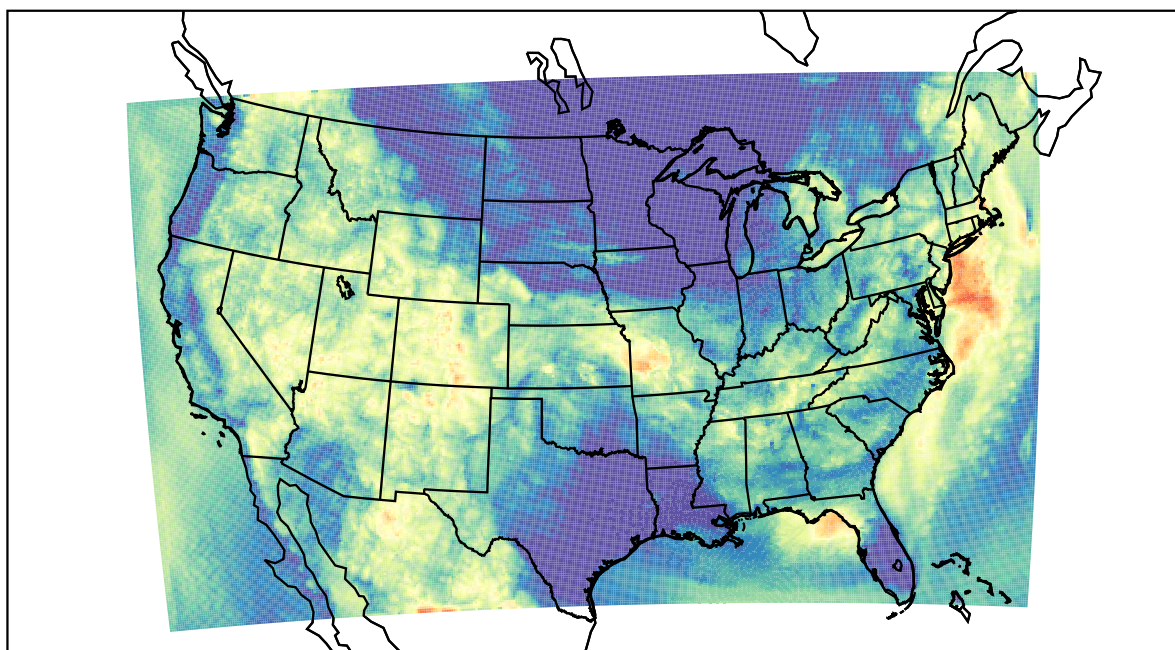
WRF (2019-08-08_11:00:00)
