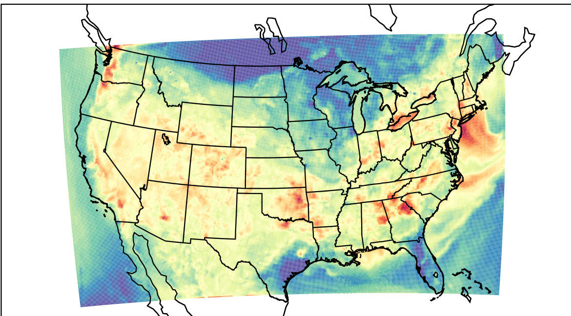
WRF (2019-08-07_02:00:00)
