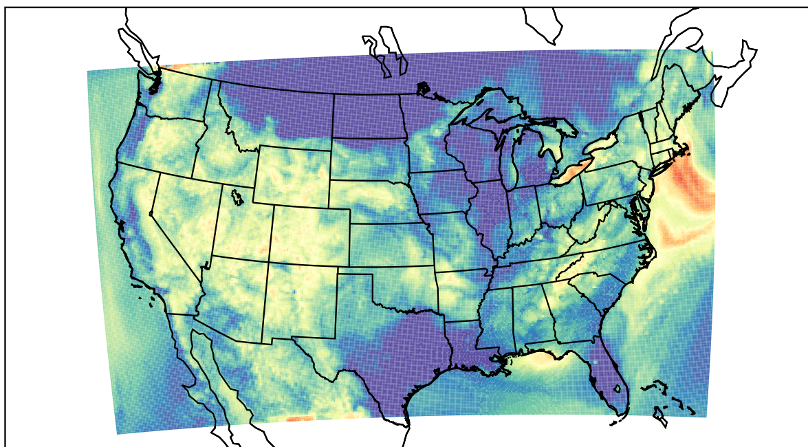
WRF (2019-08-07_12:00:00)
