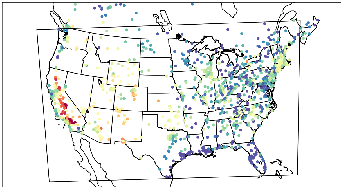
AirNOW (2019-08-08_01:00:00)
