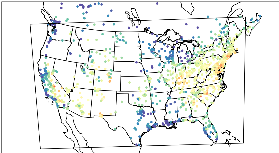
AirNOW (2019-08-08_16:00:00)
