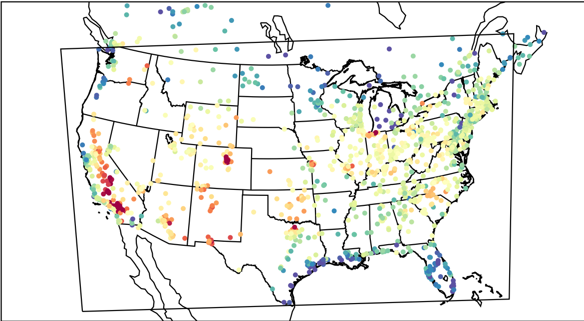
AirNOW (2019-08-07_22:00:00)
