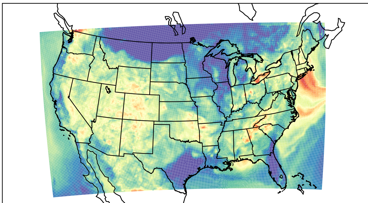
WRF (2019-08-07_07:00:00)
