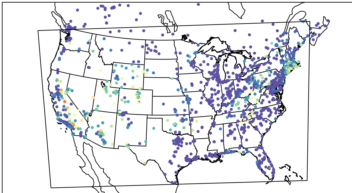
AirNOW (2019-08-07_11:00:00)
