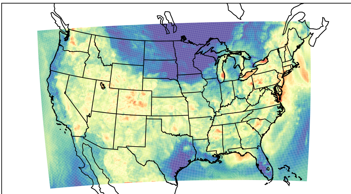
WRF (2019-08-08_04:00:00)
