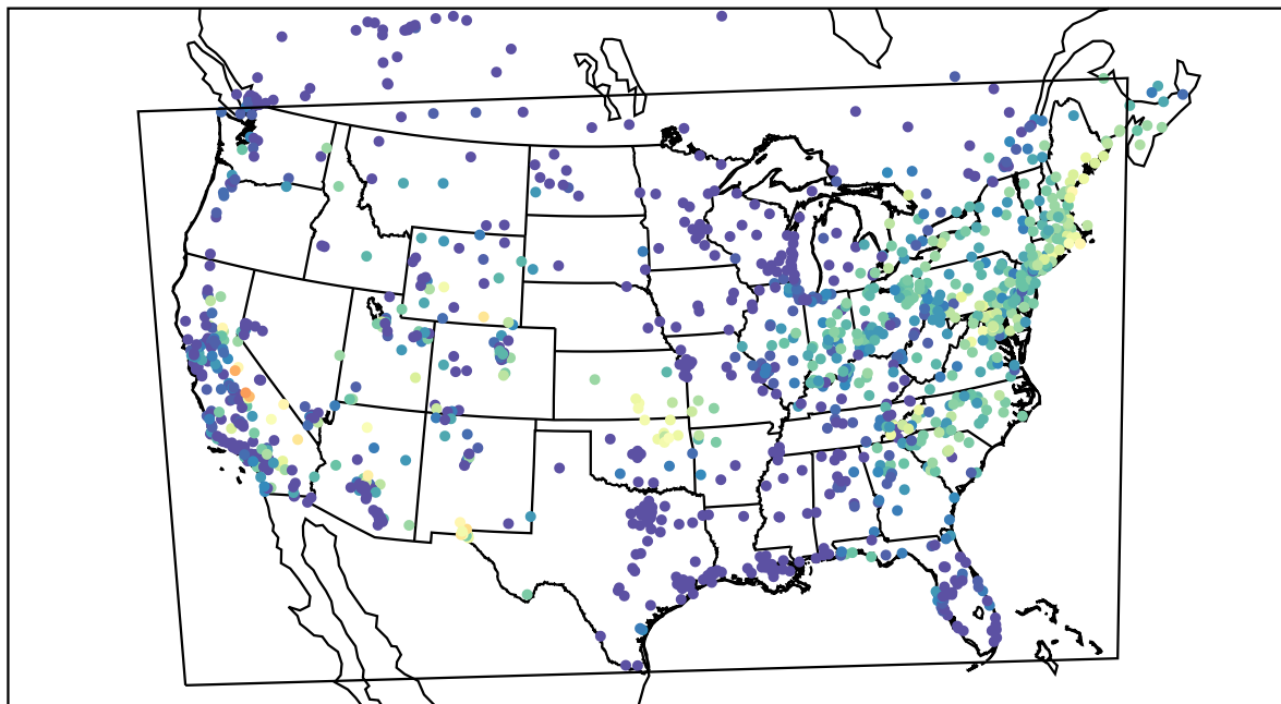
AirNOW (2019-08-08_13:00:00)
