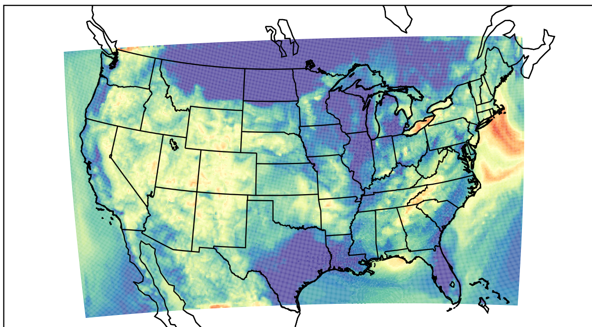
WRF (2019-08-07_11:00:00)
