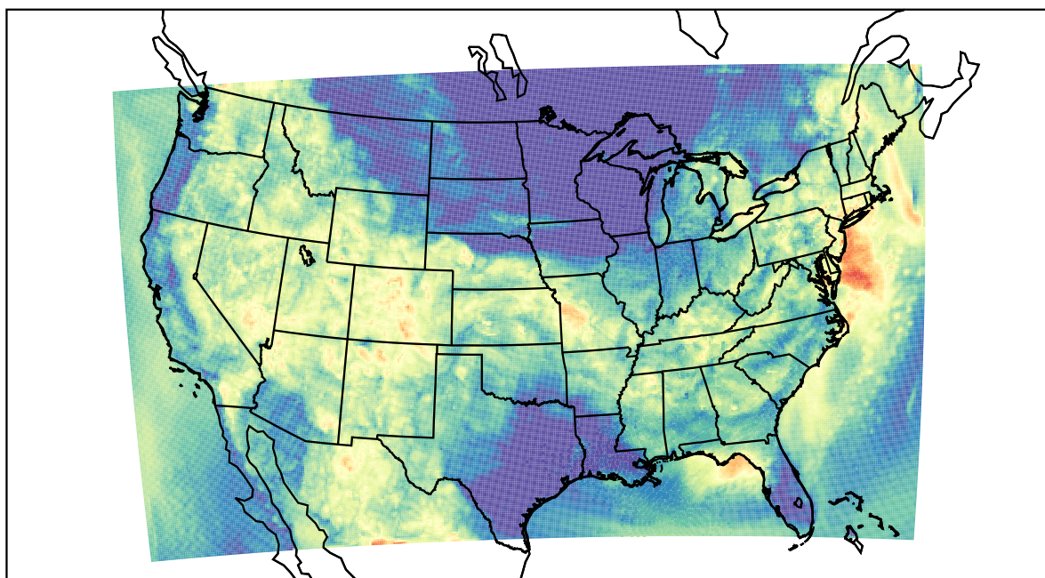
WRF (2019-08-08_09:00:00)
