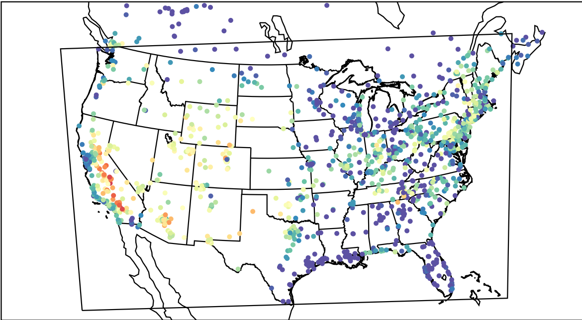
AirNOW (2019-08-07_03:00:00)
