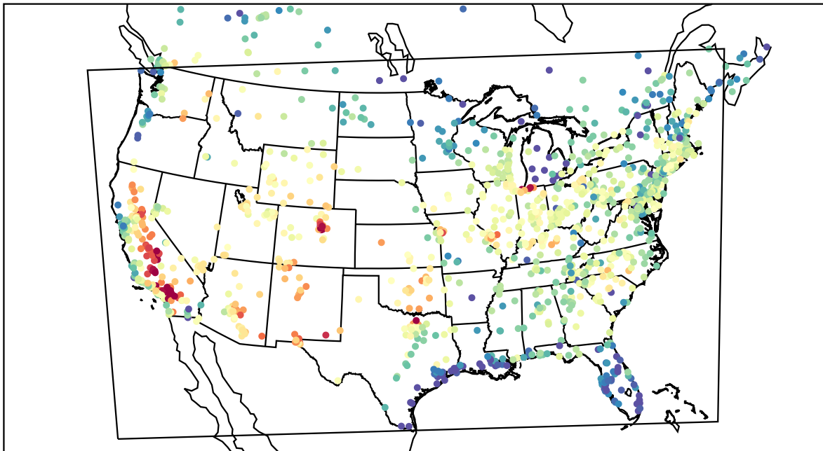
AirNOW (2019-08-07_23:00:00)
