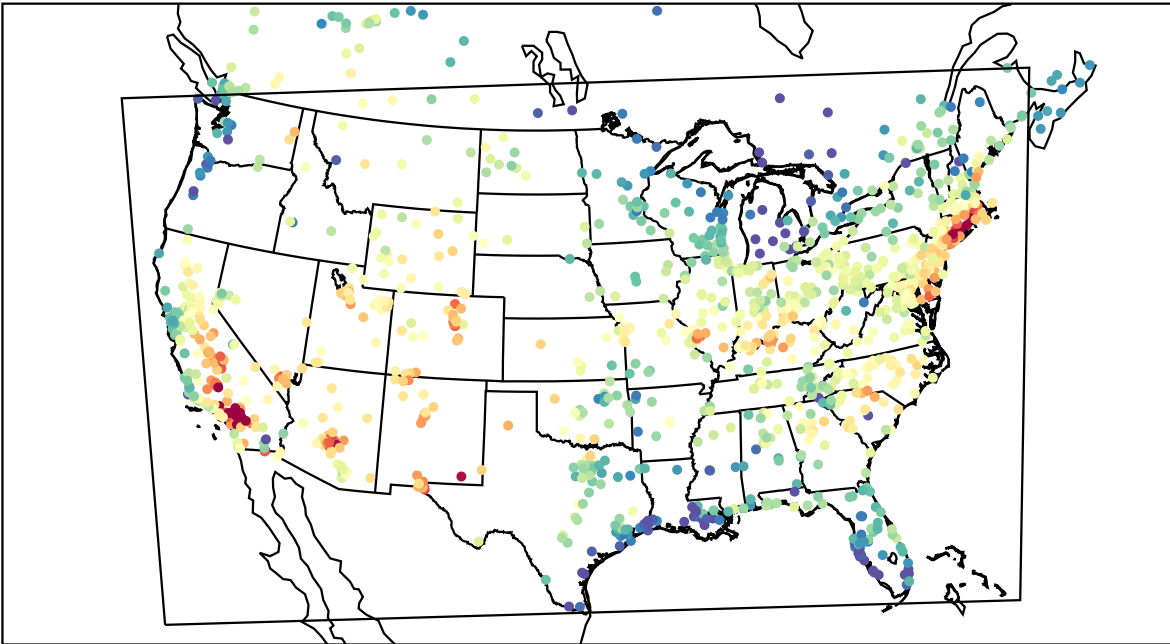
AirNOW (2019-08-08_22:00:00)
