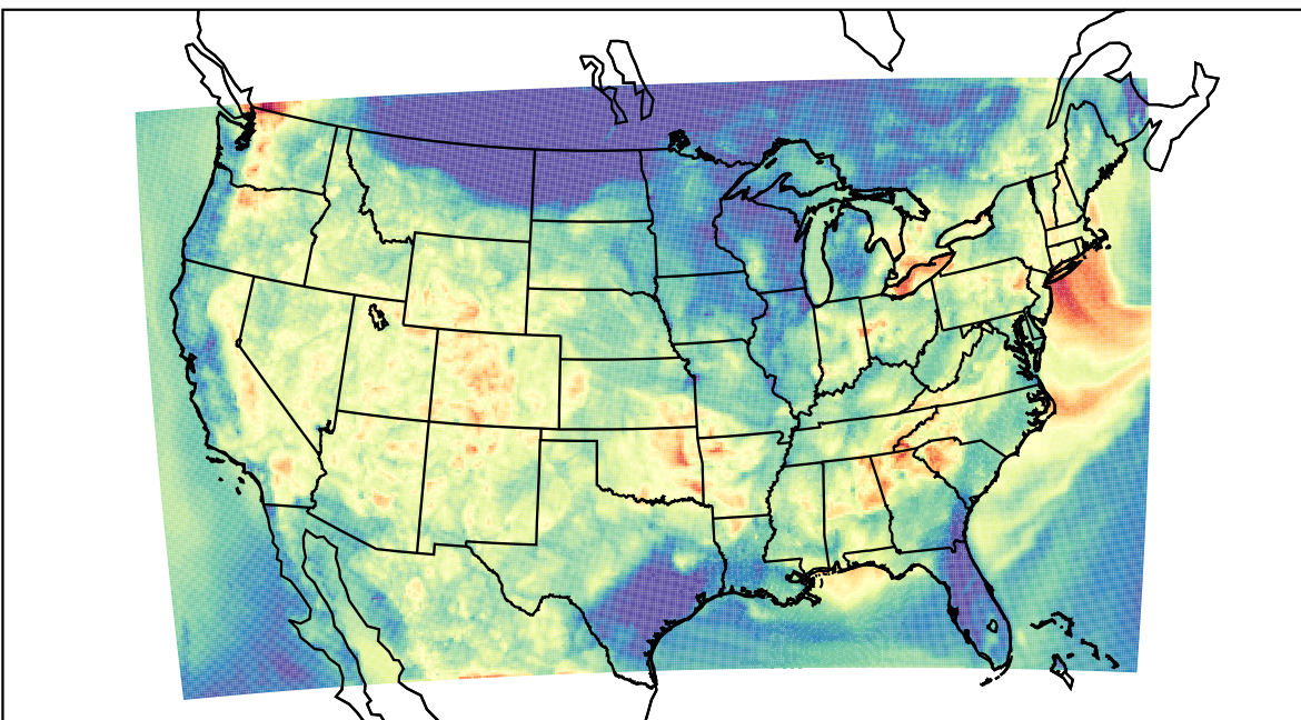
WRF (2019-08-07_05:00:00)
