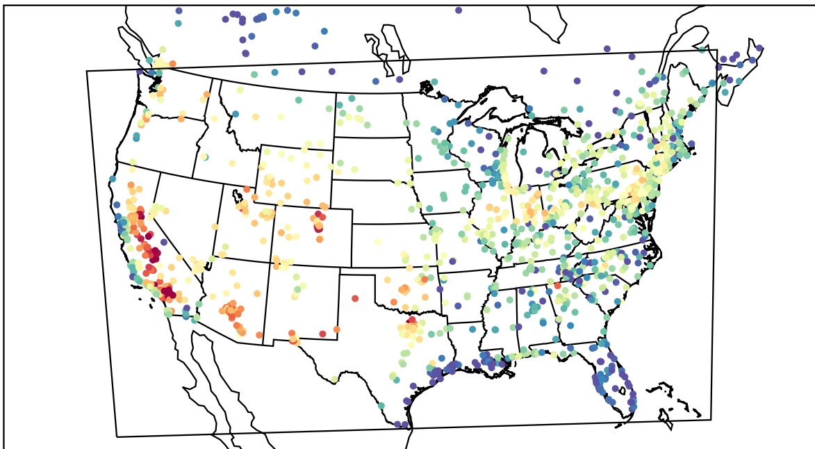
AirNOW (2019-08-07_00:00:00)
