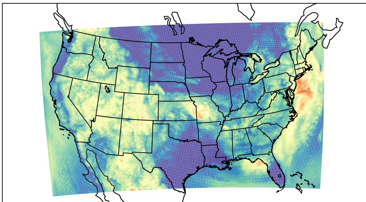
WRF (2019-08-08_12:00:00)
