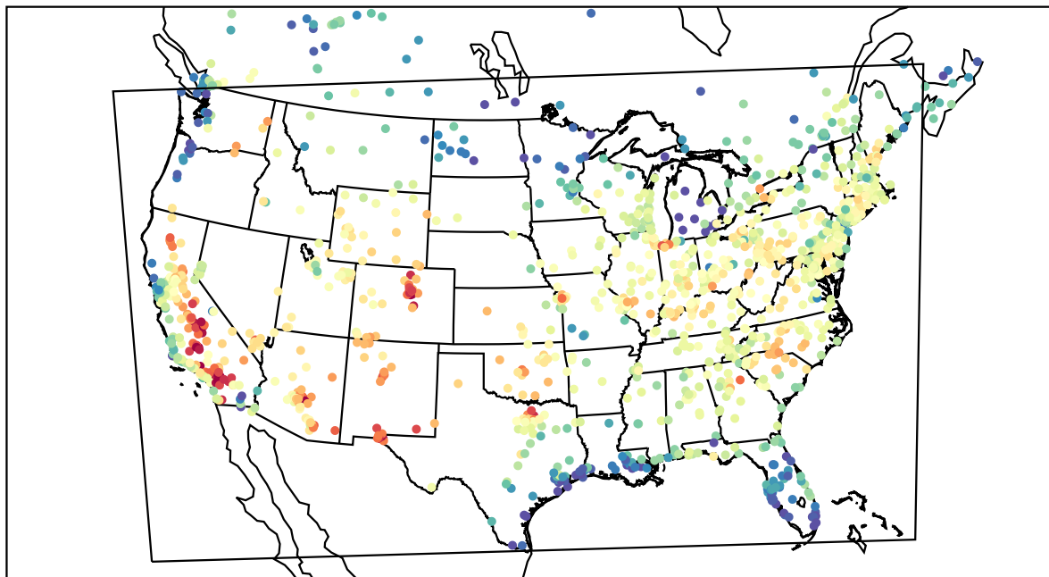
AirNOW (2019-08-07_20:00:00)
