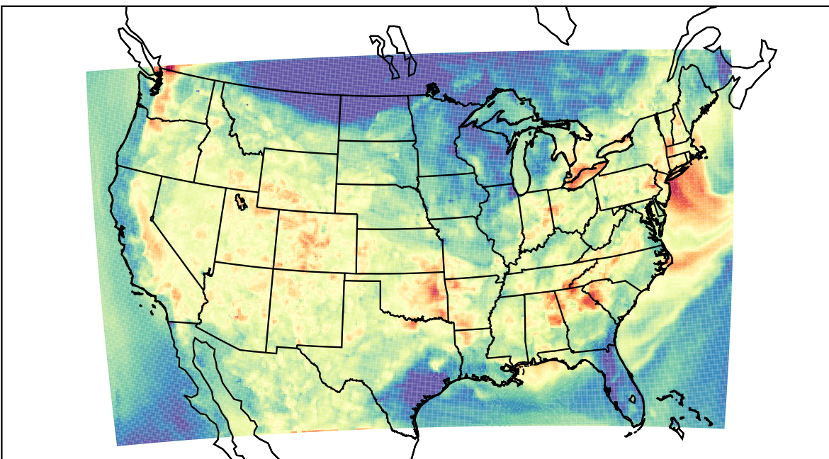
WRF (2019-08-07_03:00:00)
