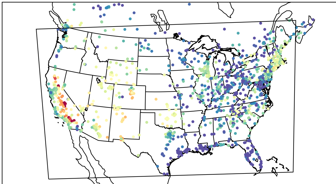
AirNOW (2019-08-08_02:00:00)
