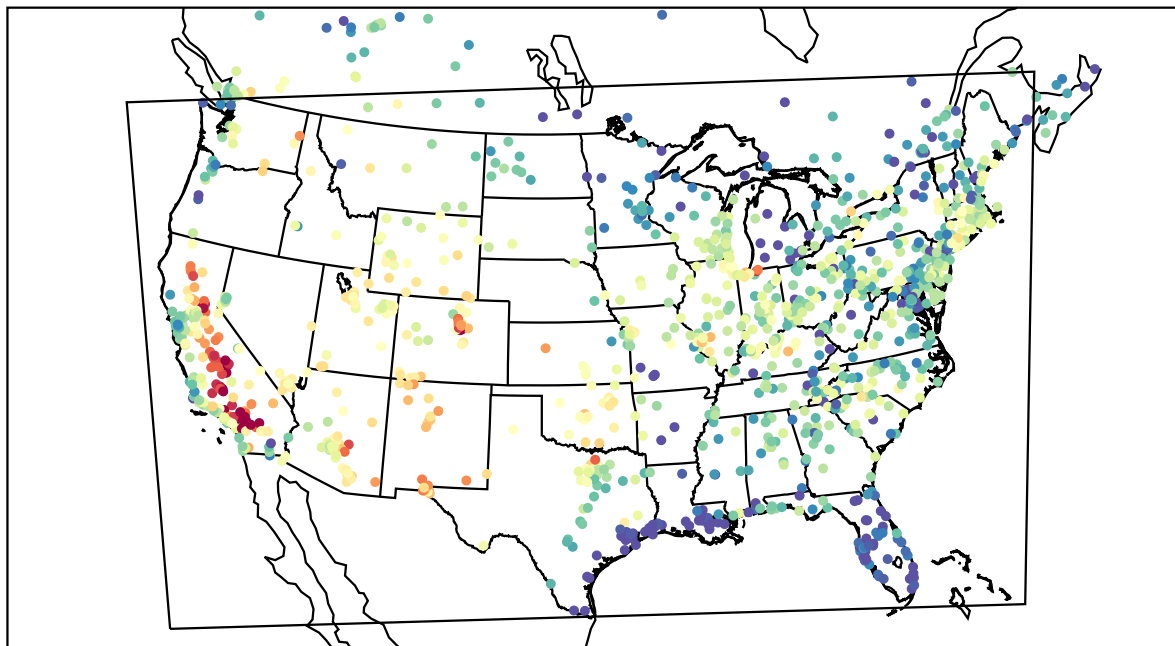
AirNOW (2019-08-08_00:00:00)
