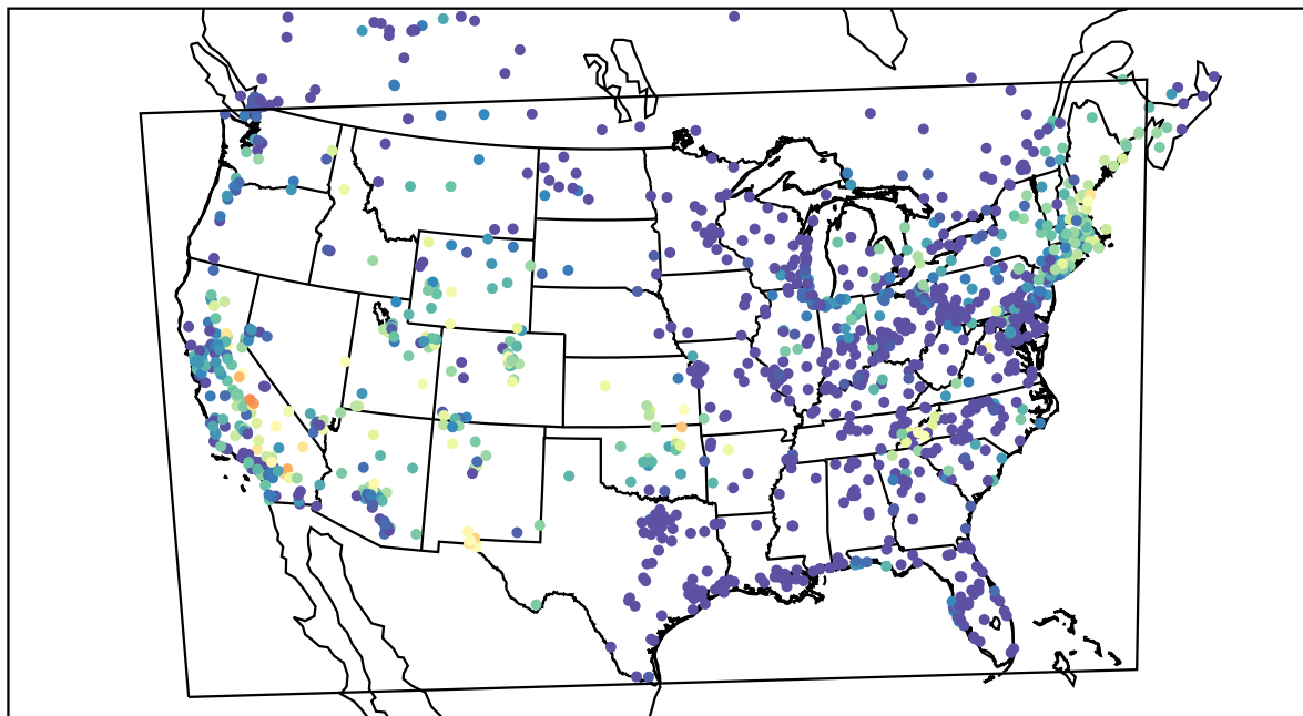
AirNOW (2019-08-08_09:00:00)
