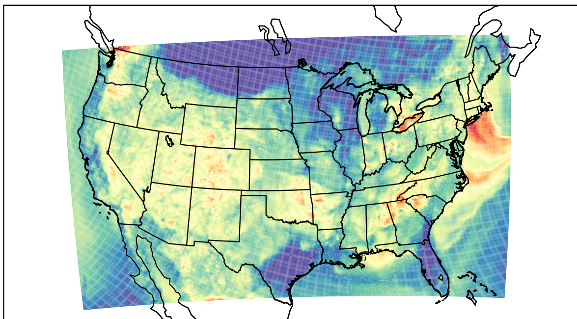
WRF (2019-08-07_06:00:00)
