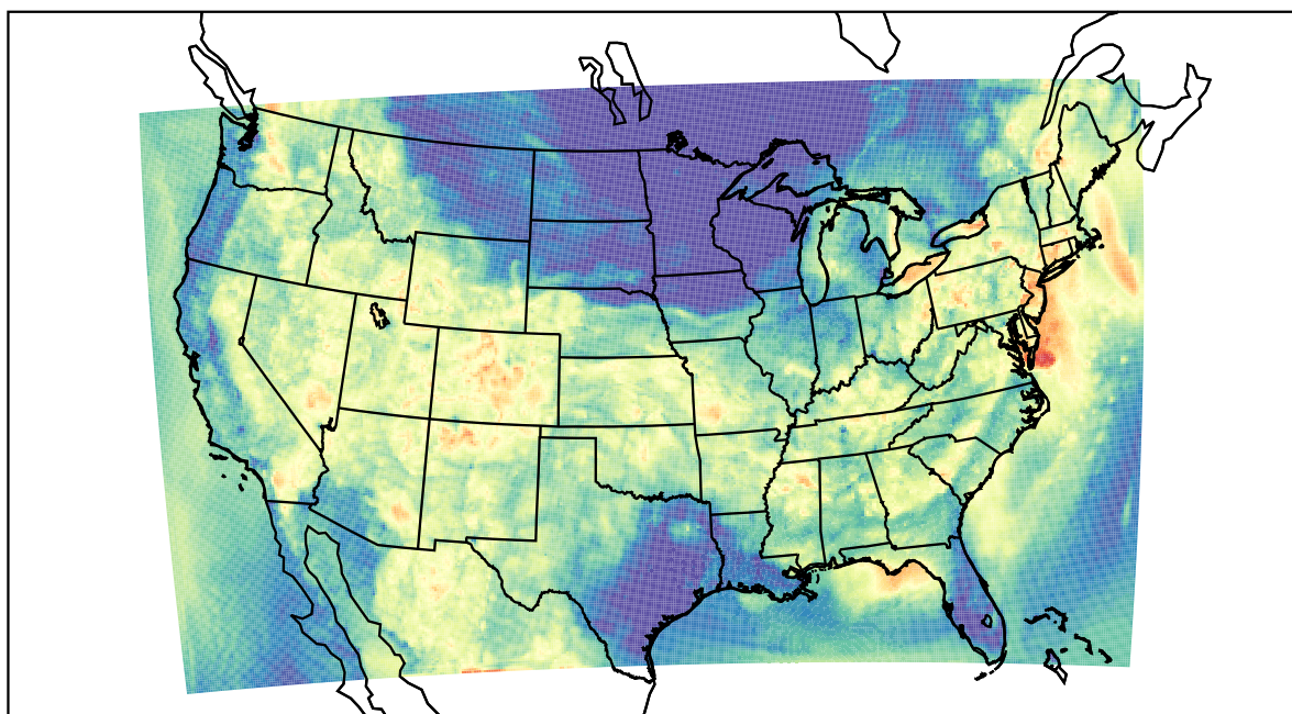
WRF (2019-08-08_06:00:00)
