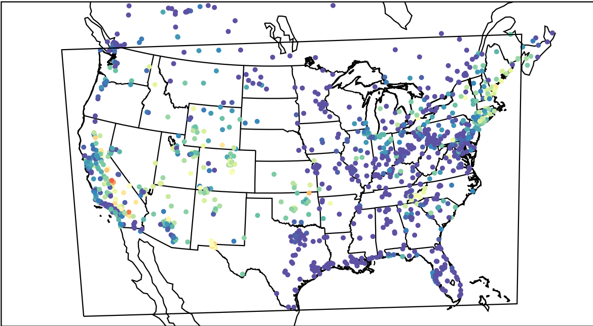
AirNOW (2019-08-08_08:00:00)
