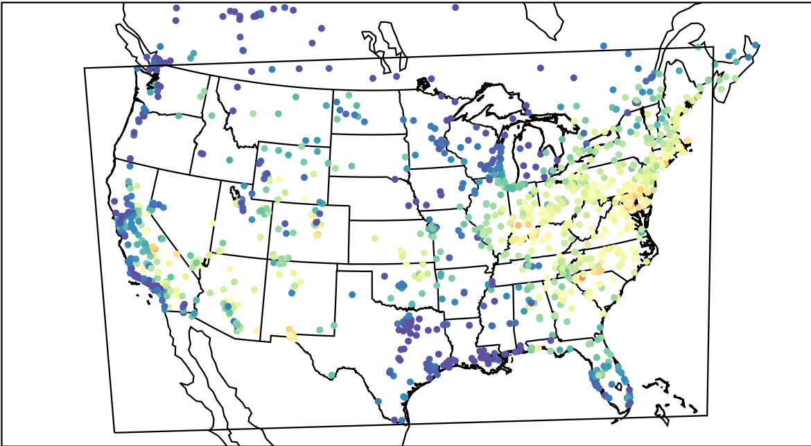
AirNOW (2019-08-08_15:00:00)
