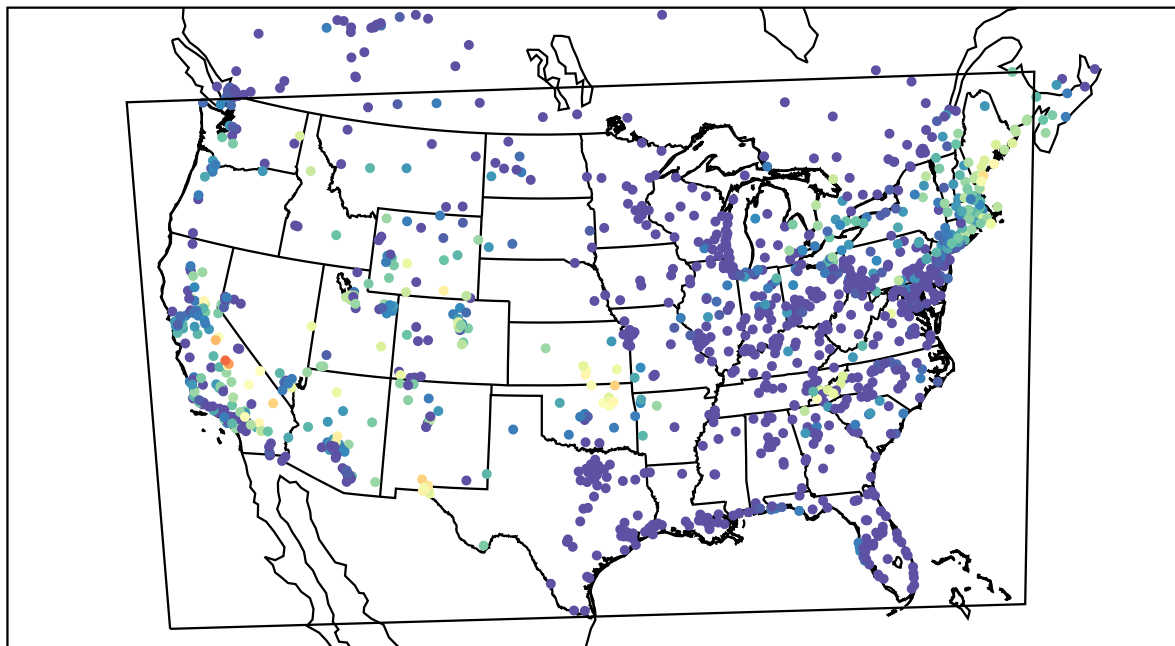
AirNOW (2019-08-08_11:00:00)
