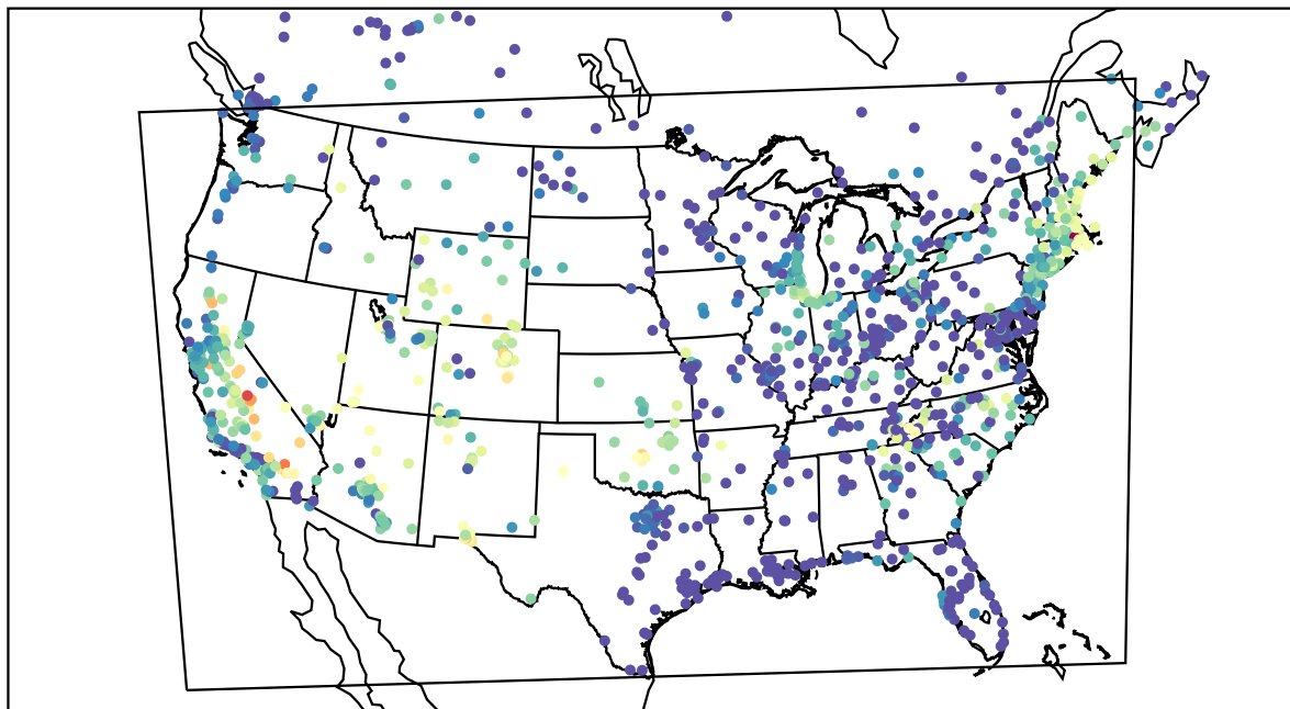
AirNOW (2019-08-08_06:00:00)
