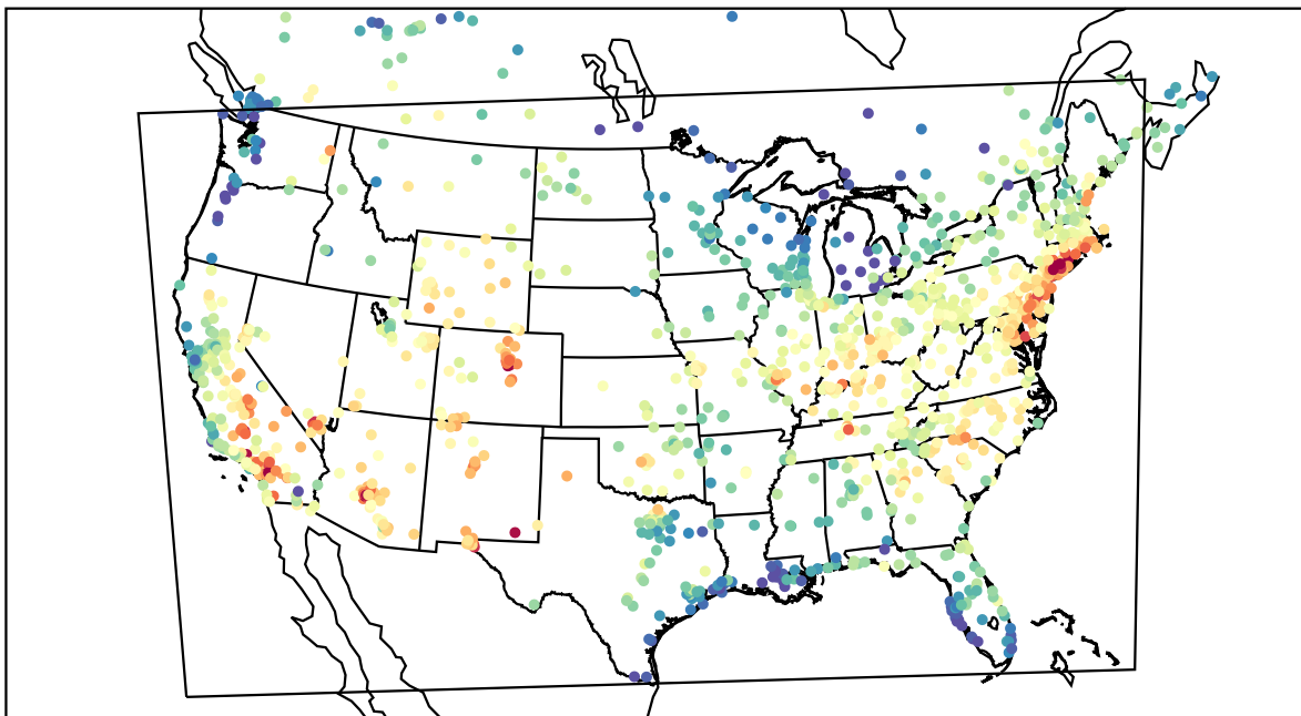
AirNOW (2019-08-08_19:00:00)
