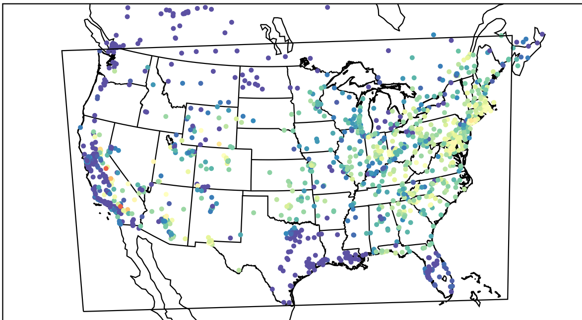
AirNOW (2019-08-07_14:00:00)
