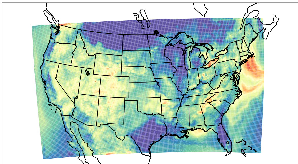
WRF (2019-08-07_09:00:00)
