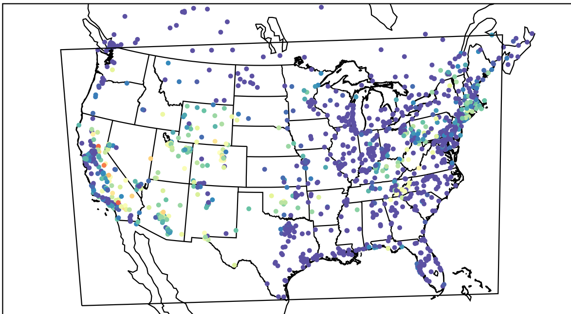
AirNOW (2019-08-07_10:00:00)
