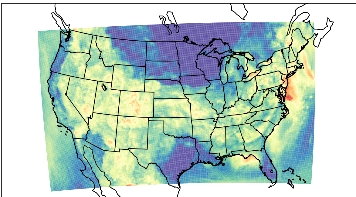
WRF (2019-08-08_07:00:00)
