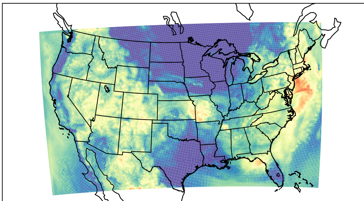
WRF (2019-08-08_13:00:00)
