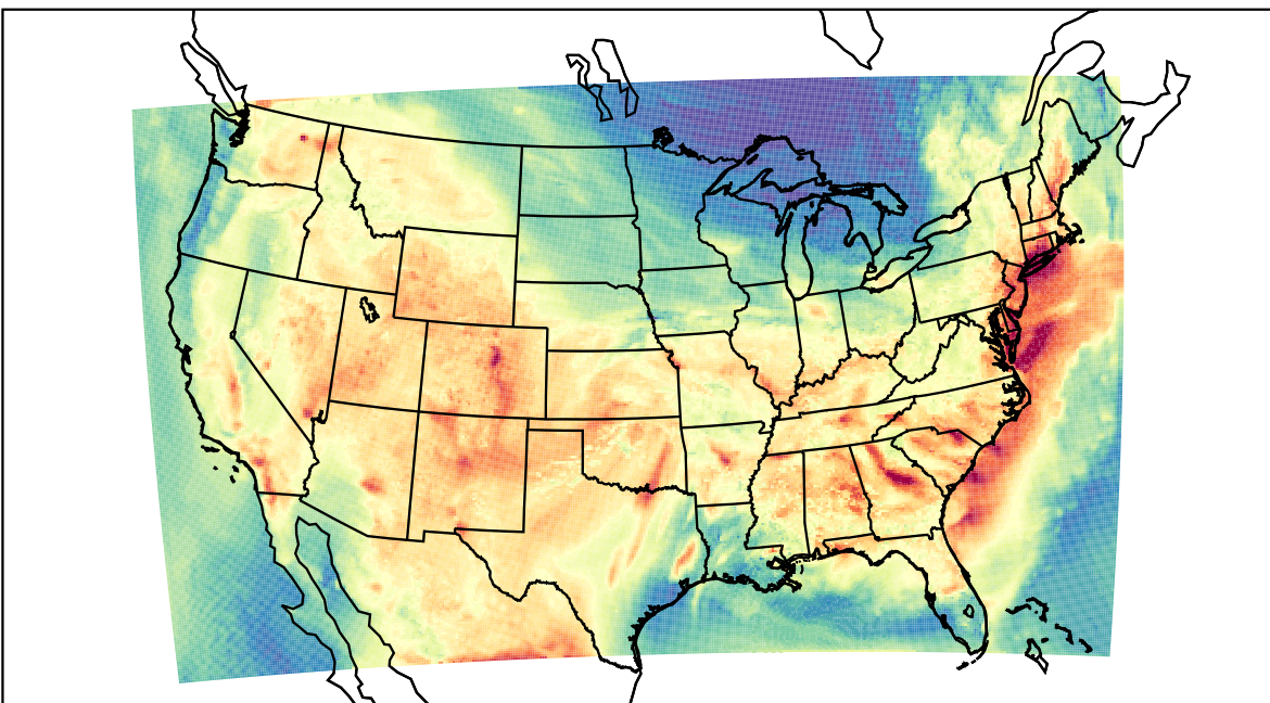
WRF (2019-08-08_22:00:00)
