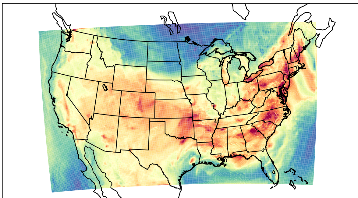
WRF (2019-08-07_20:00:00)
