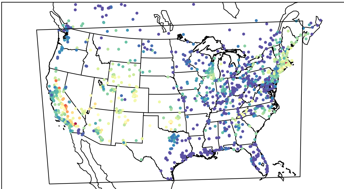
AirNOW (2019-08-08_04:00:00)
