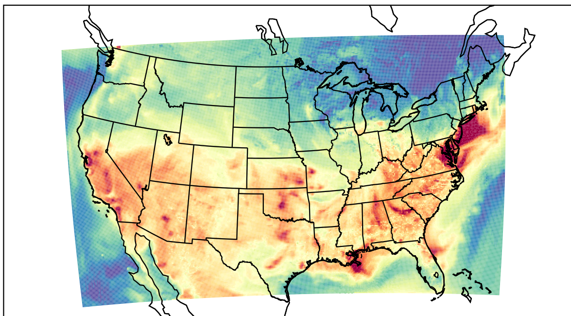
WRF (2019-08-14_22:00:00)
