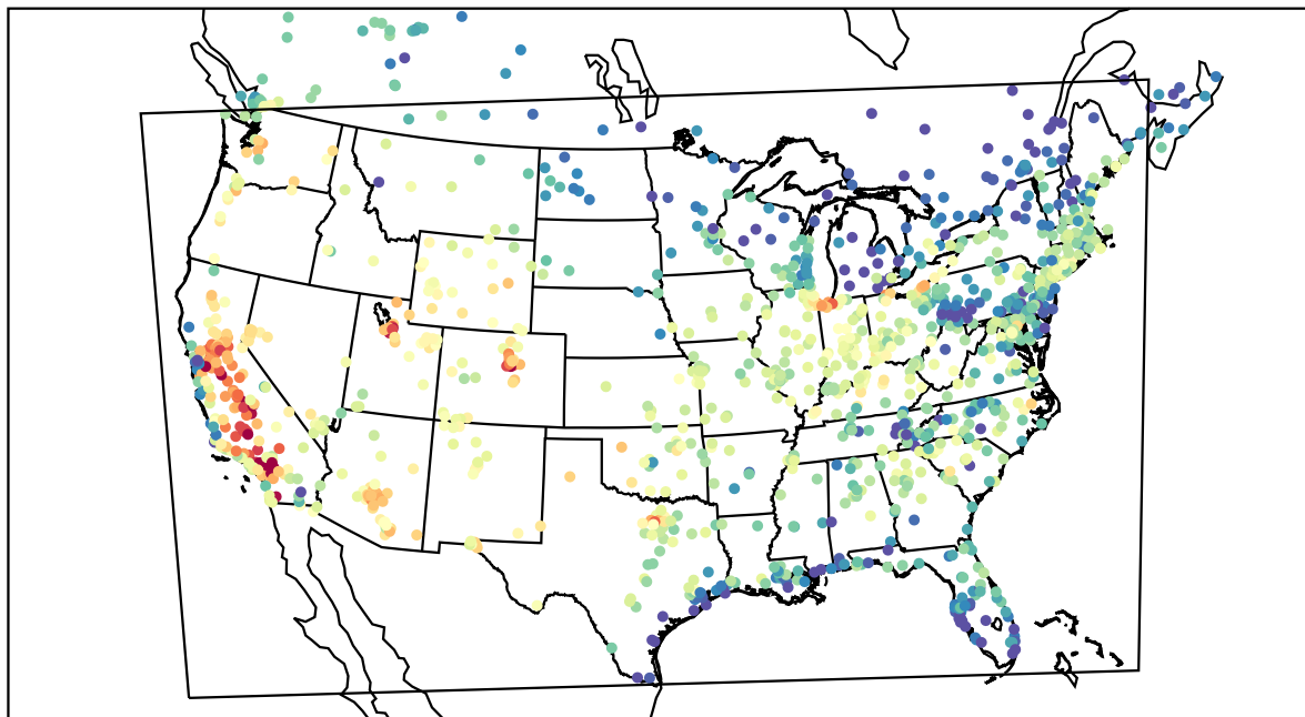
AirNOW (2019-08-13_23:00:00)
