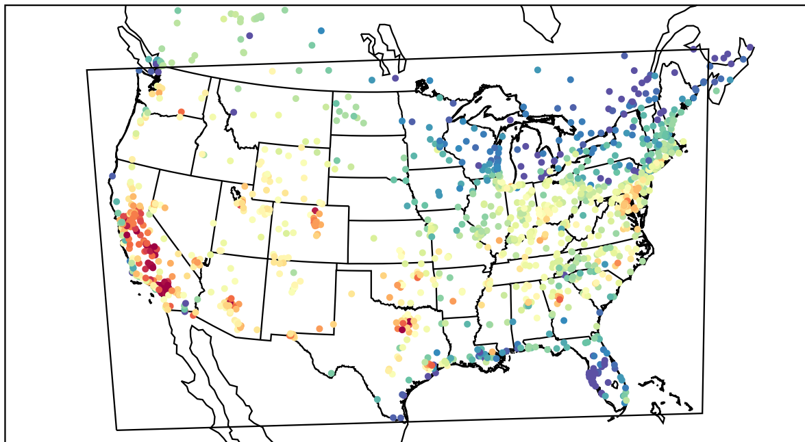
AirNOW (2019-08-14_22:00:00)
