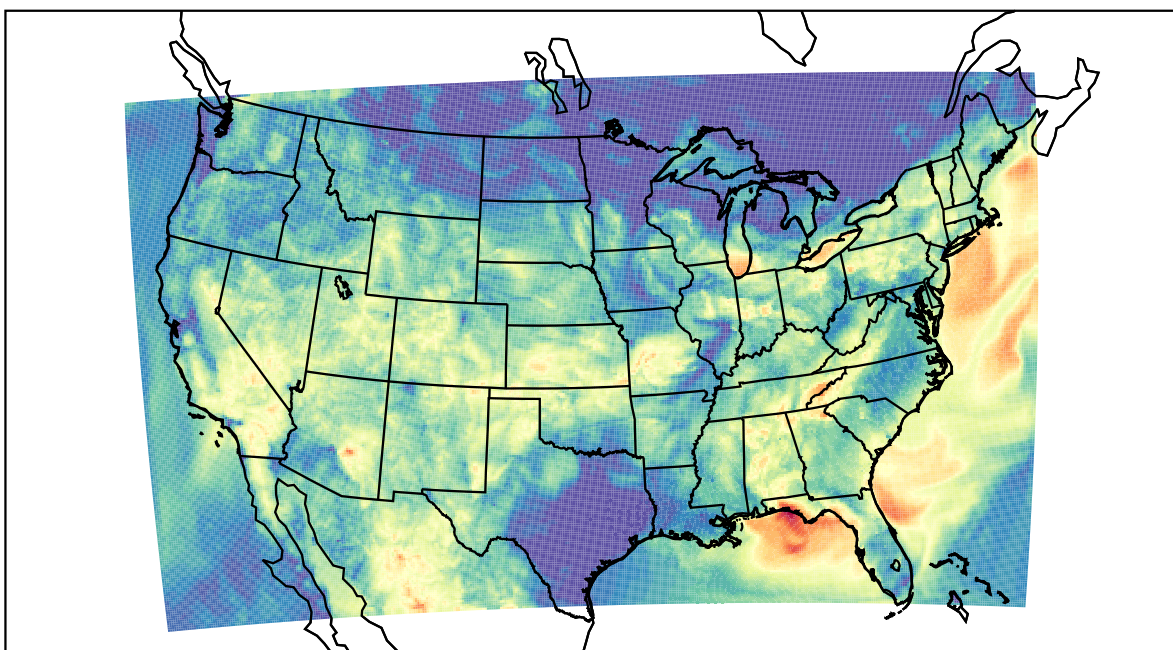
WRF (2019-08-13_08:00:00)
