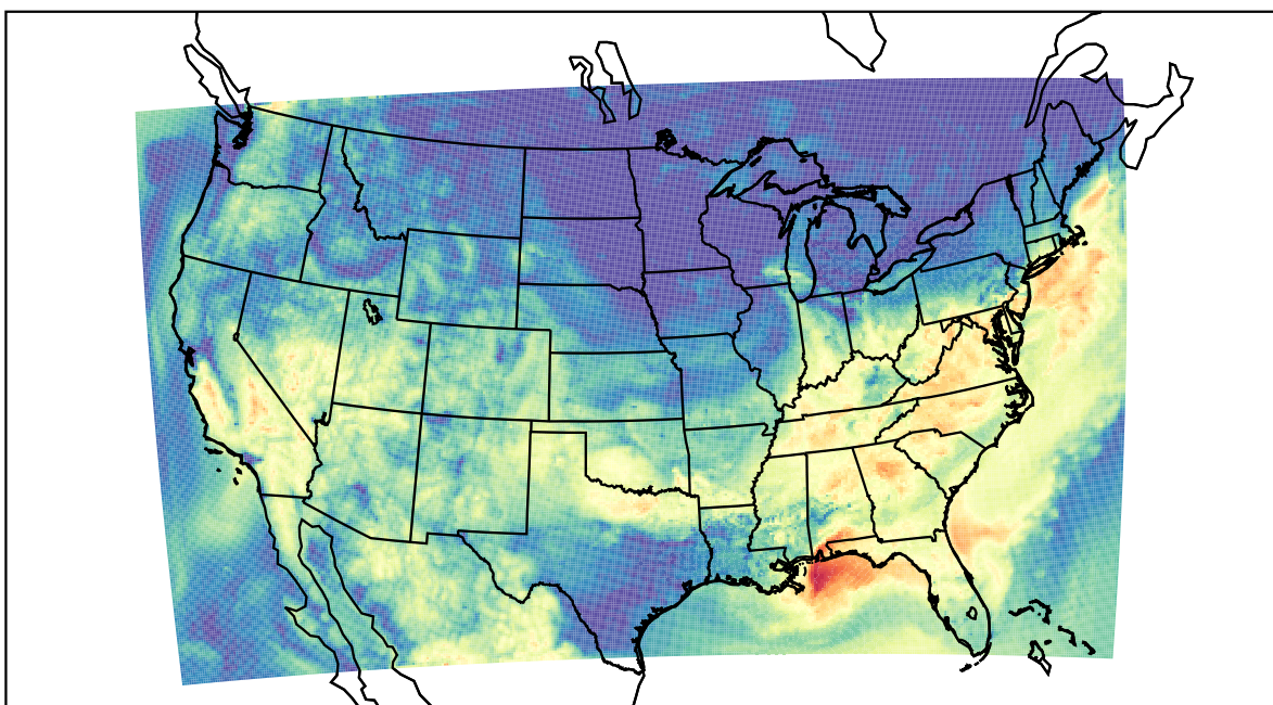
WRF (2019-08-14_14:00:00)
