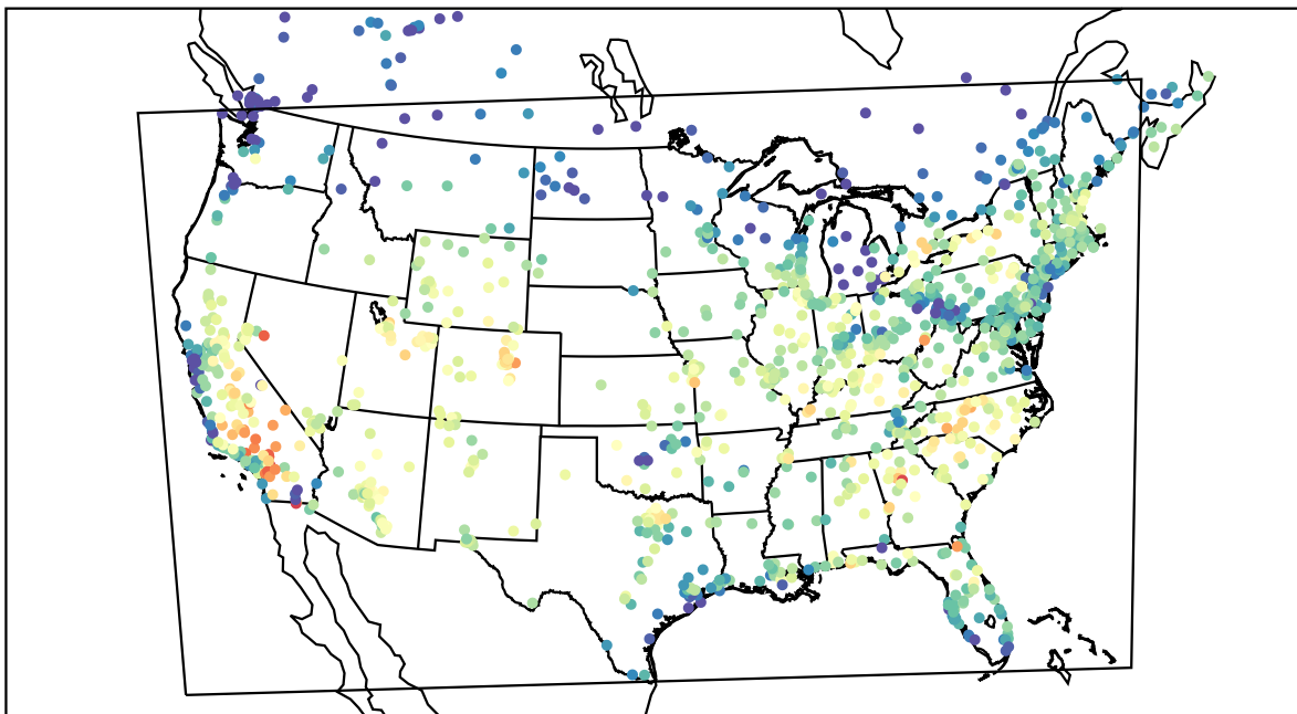
AirNOW (2019-08-13_17:00:00)
