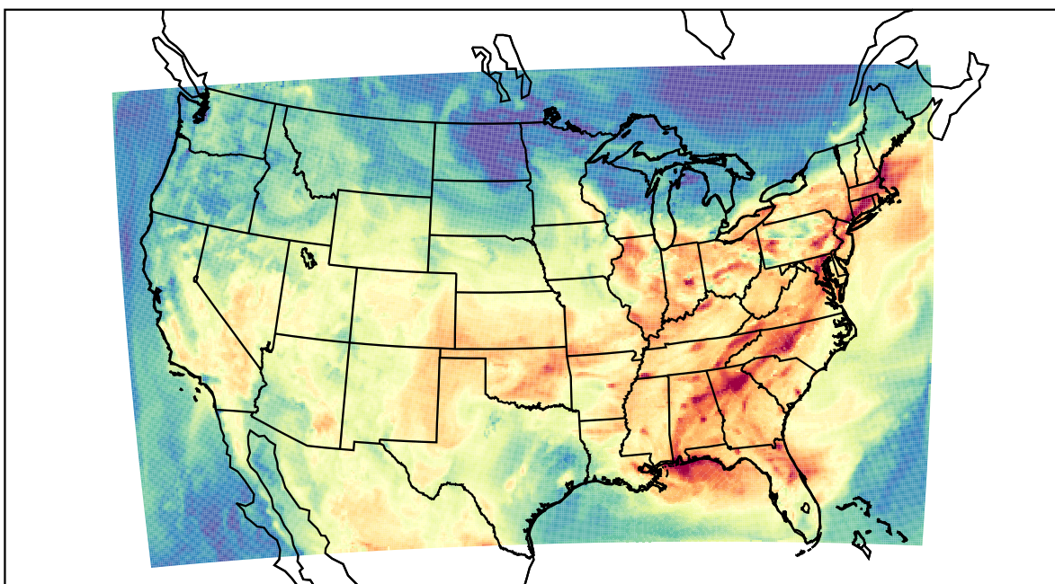
WRF (2019-08-13_17:00:00)
