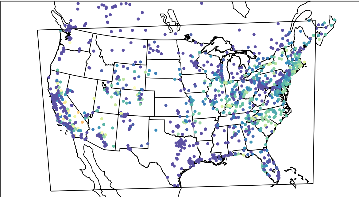
AirNOW (2019-08-13_13:00:00)
