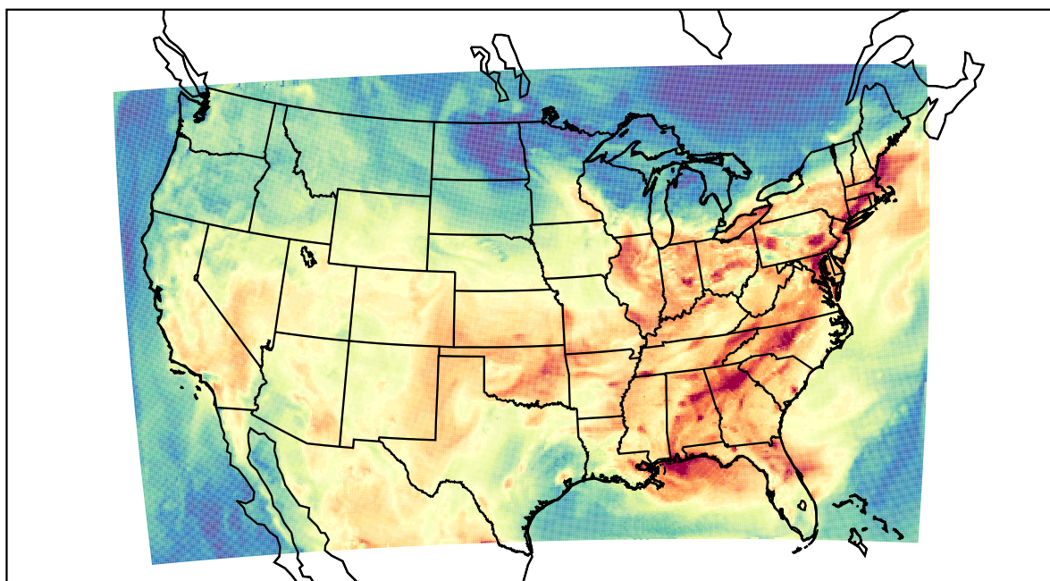
WRF (2019-08-13_18:00:00)
