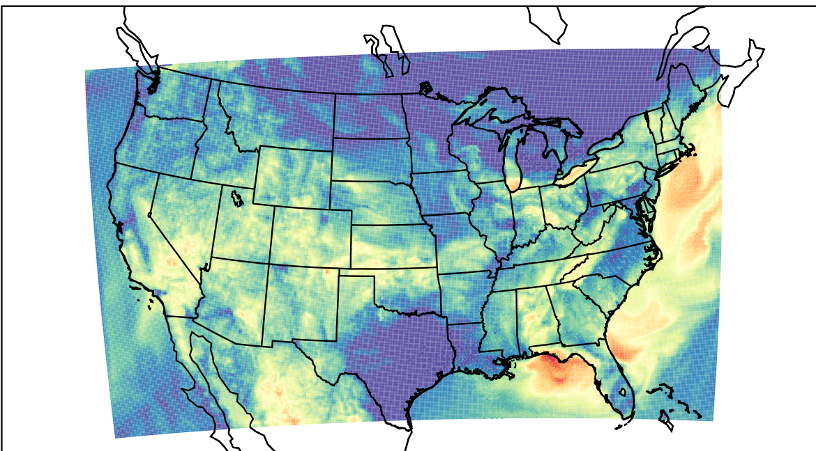
WRF (2019-08-13_11:00:00)
