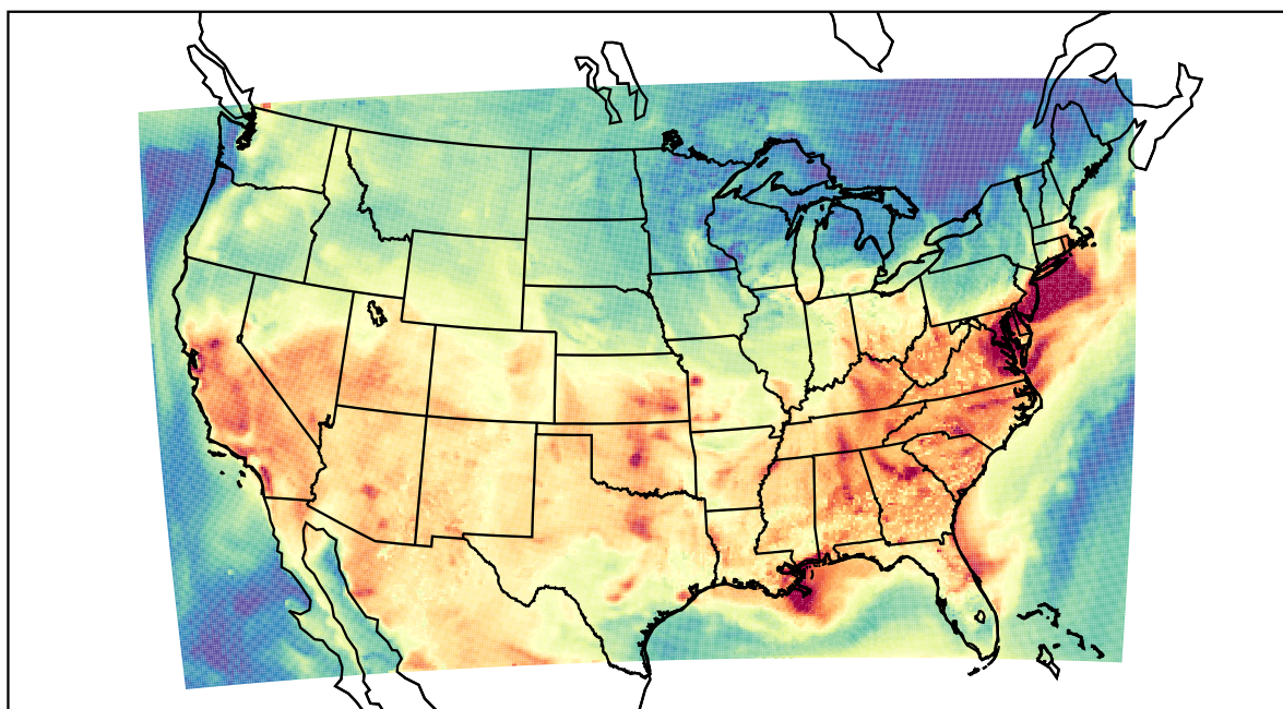
WRF (2019-08-14_20:00:00)
