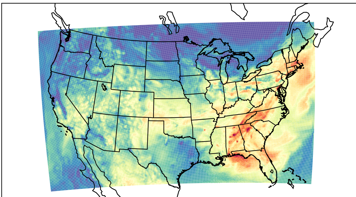
WRF (2019-08-13_15:00:00)
