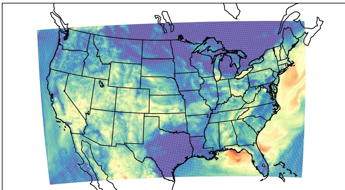
WRF (2019-08-13_12:00:00)
