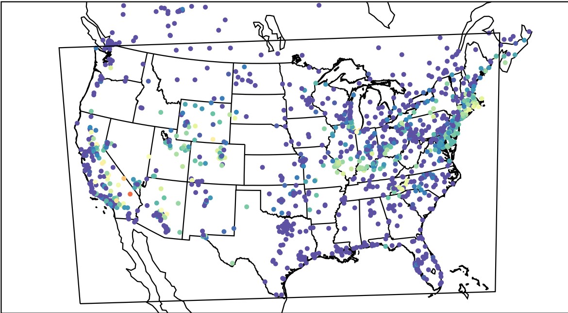
AirNOW (2019-08-13_11:00:00)
