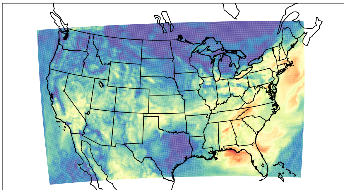
WRF (2019-08-13_14:00:00)
