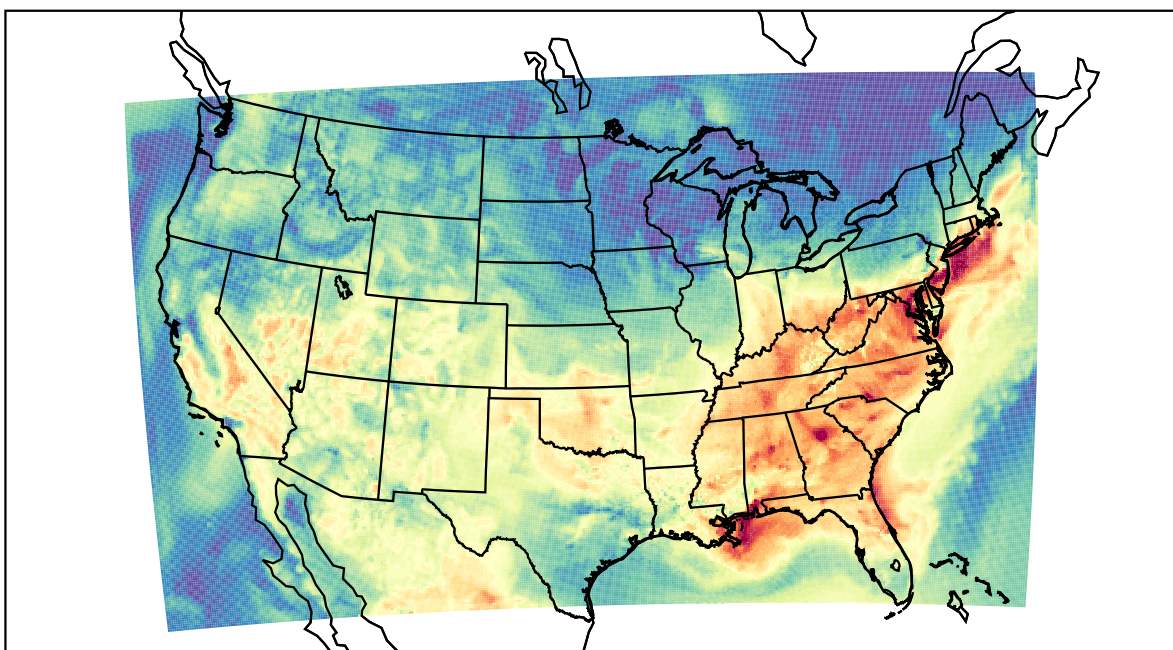
WRF (2019-08-14_16:00:00)
