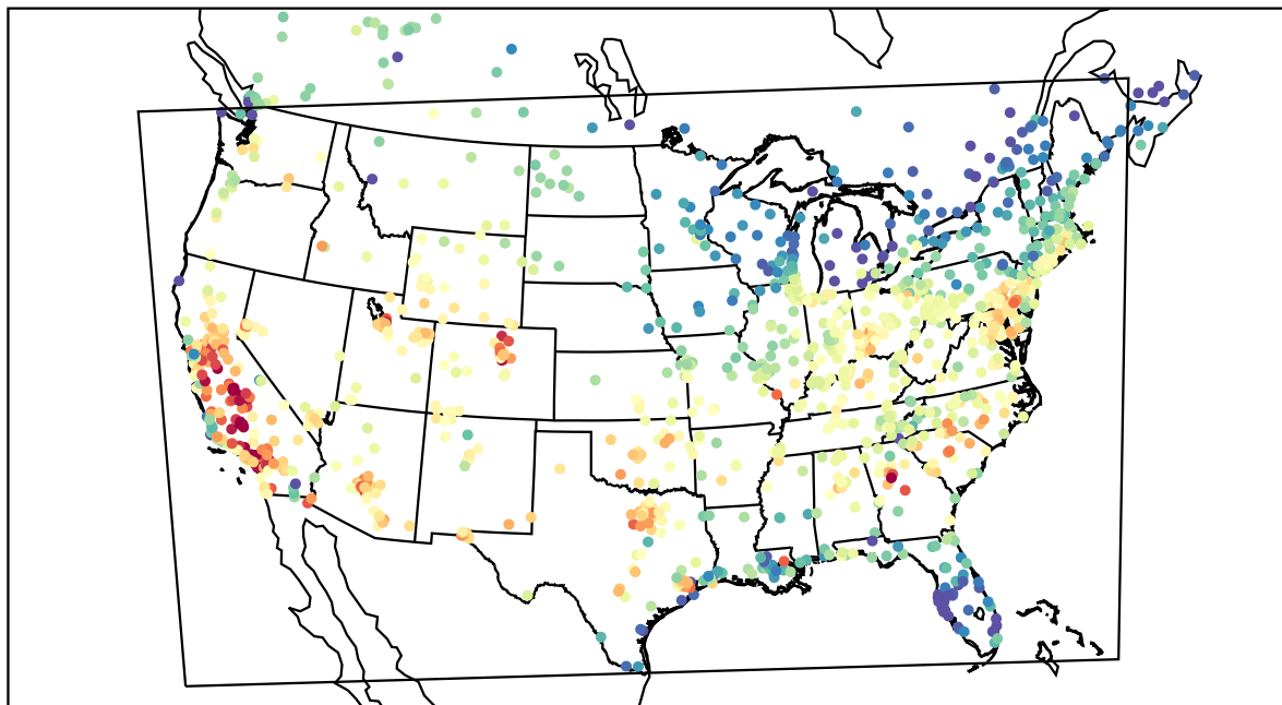
AirNOW (2019-08-14_20:00:00)
