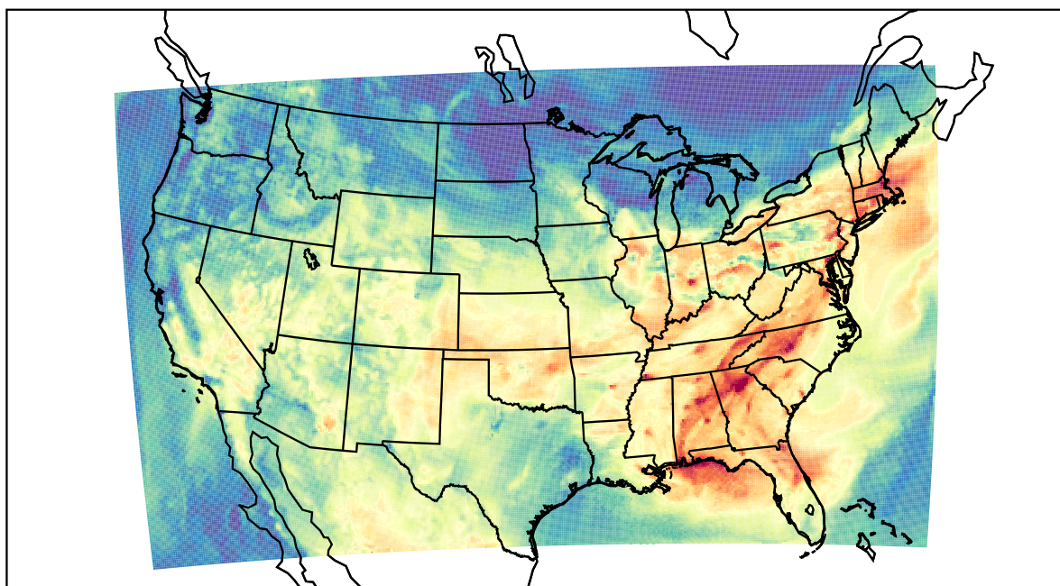
WRF (2019-08-13_16:00:00)
