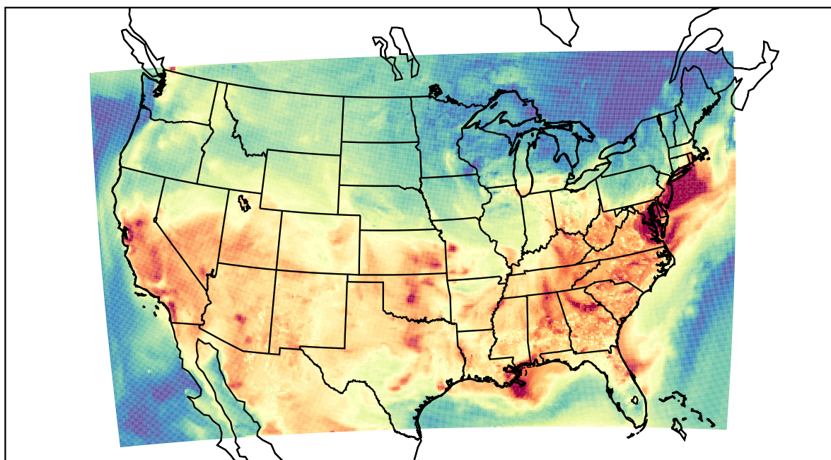
WRF (2019-08-14_21:00:00)
