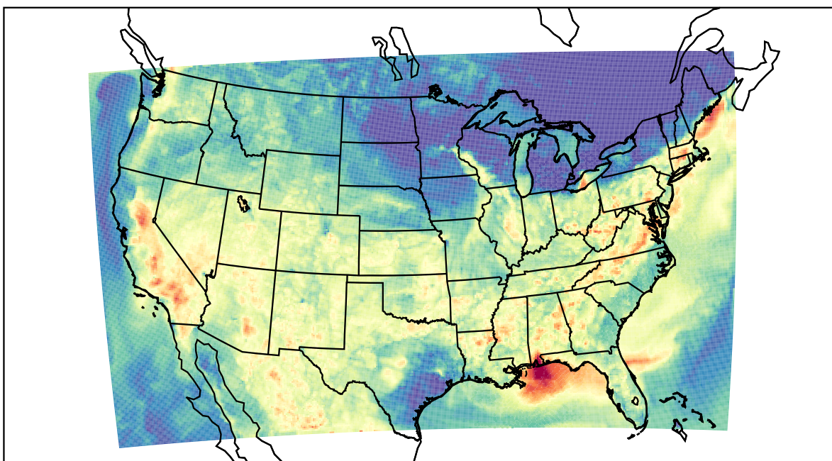
WRF (2019-08-14_03:00:00)
