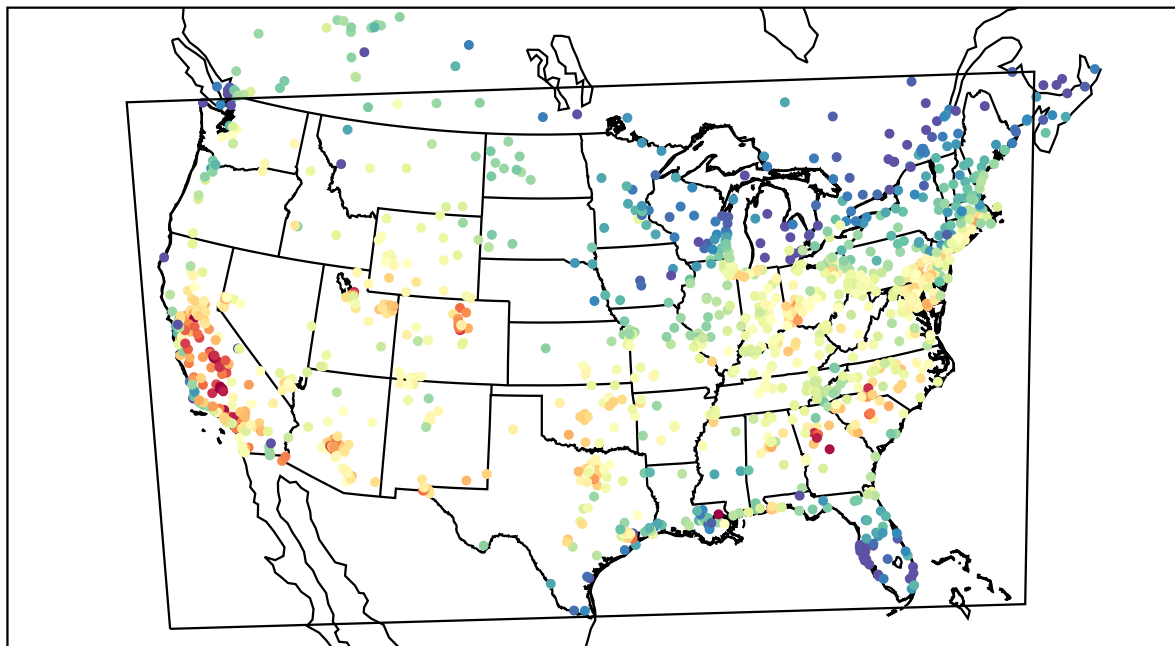
AirNOW (2019-08-14_19:00:00)
