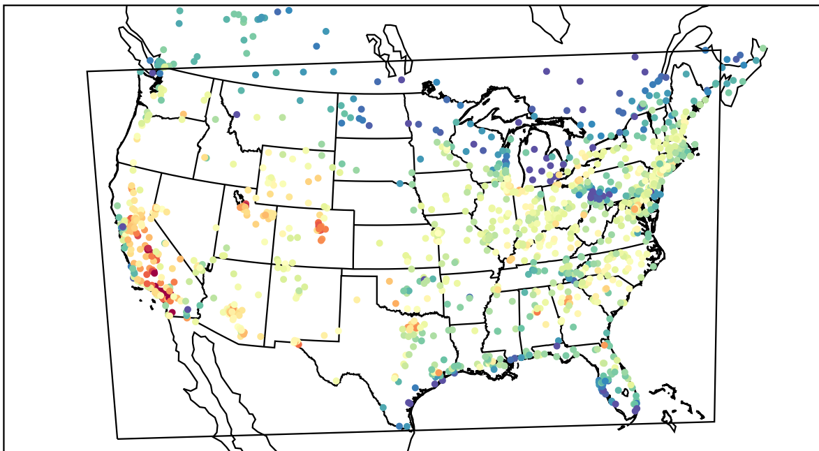
AirNOW (2019-08-13_20:00:00)
