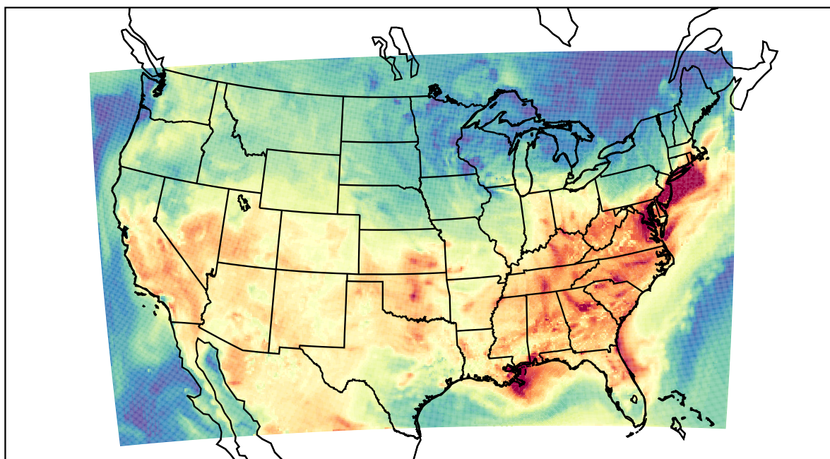
WRF (2019-08-14_18:00:00)
