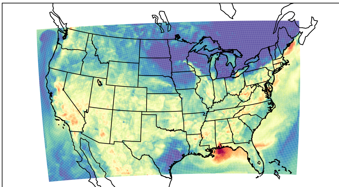
WRF (2019-08-14_04:00:00)
