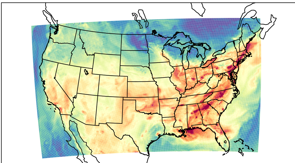
WRF (2019-08-13_19:00:00)
