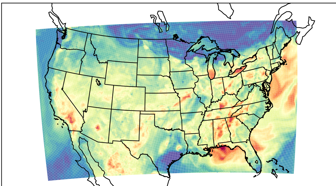
WRF (2019-08-13_02:00:00)
