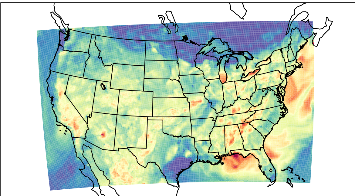
WRF (2019-08-13_03:00:00)
