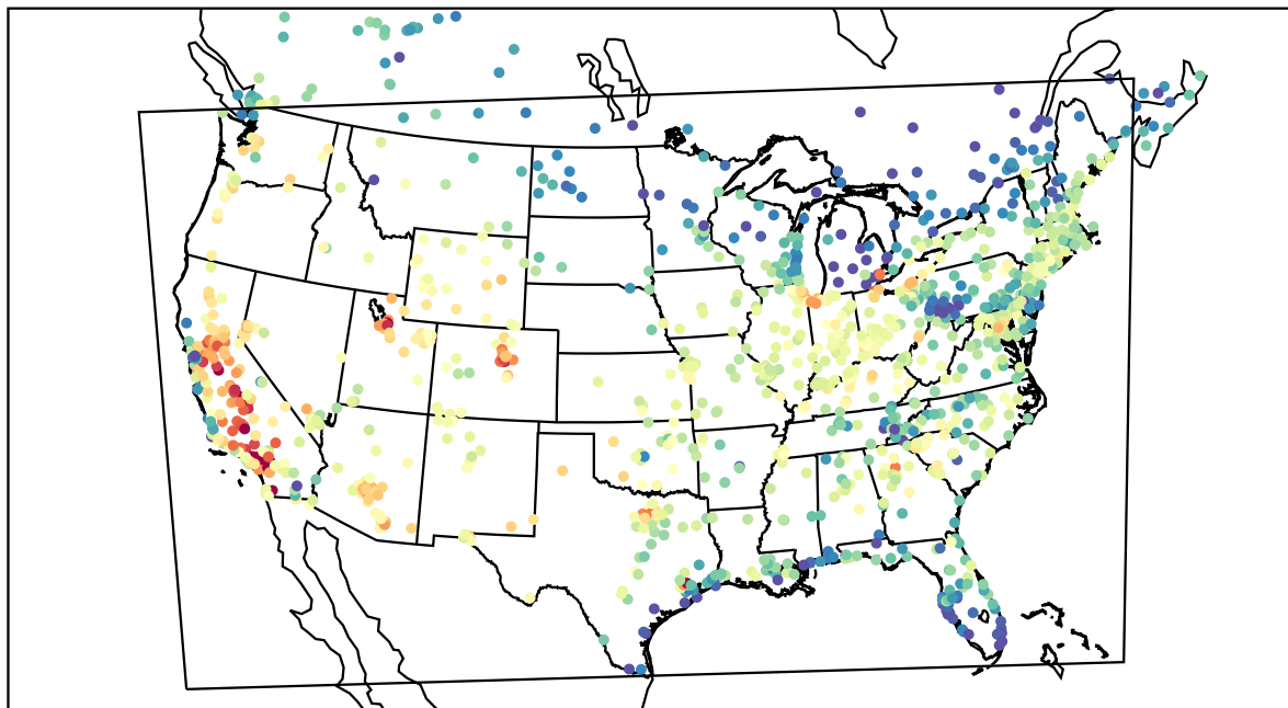
AirNOW (2019-08-13_22:00:00)
