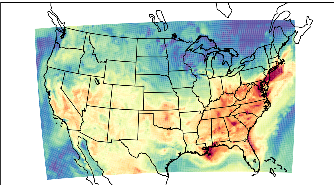
WRF (2019-08-14_17:00:00)
