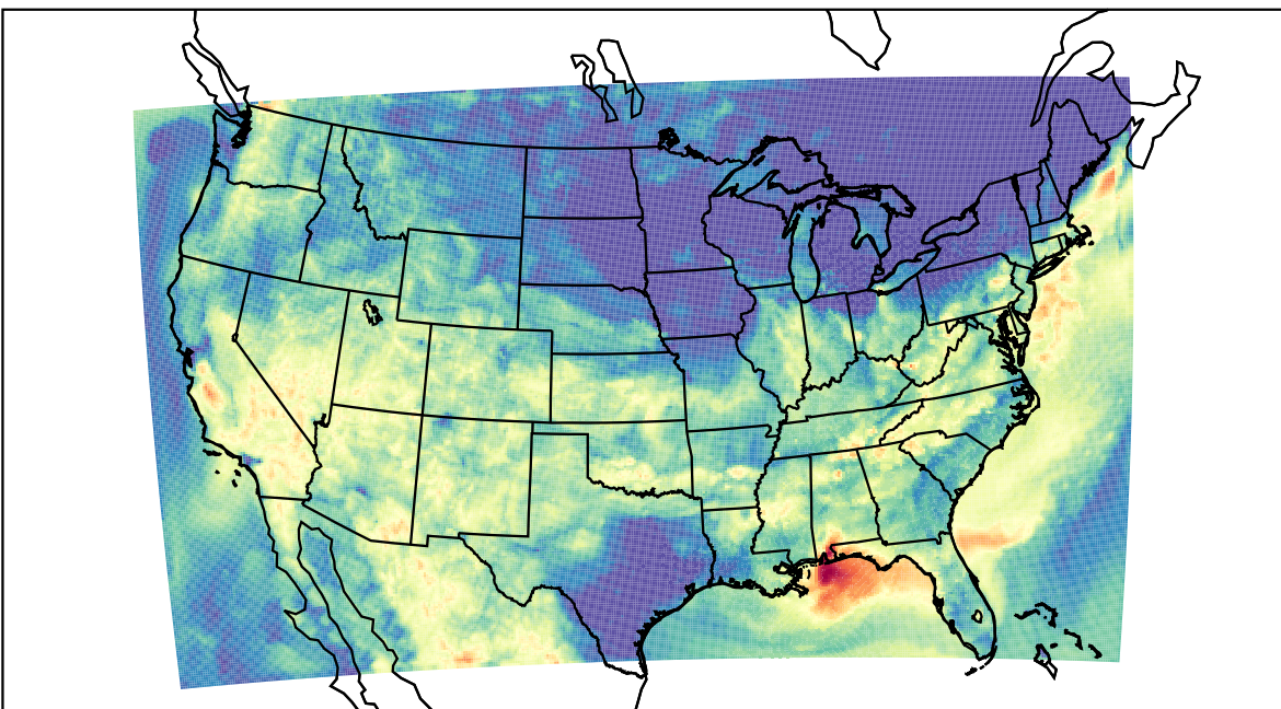
WRF (2019-08-14_08:00:00)
