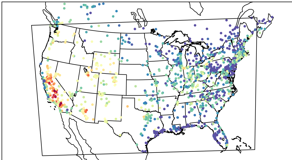
AirNOW (2019-08-14_01:00:00)
