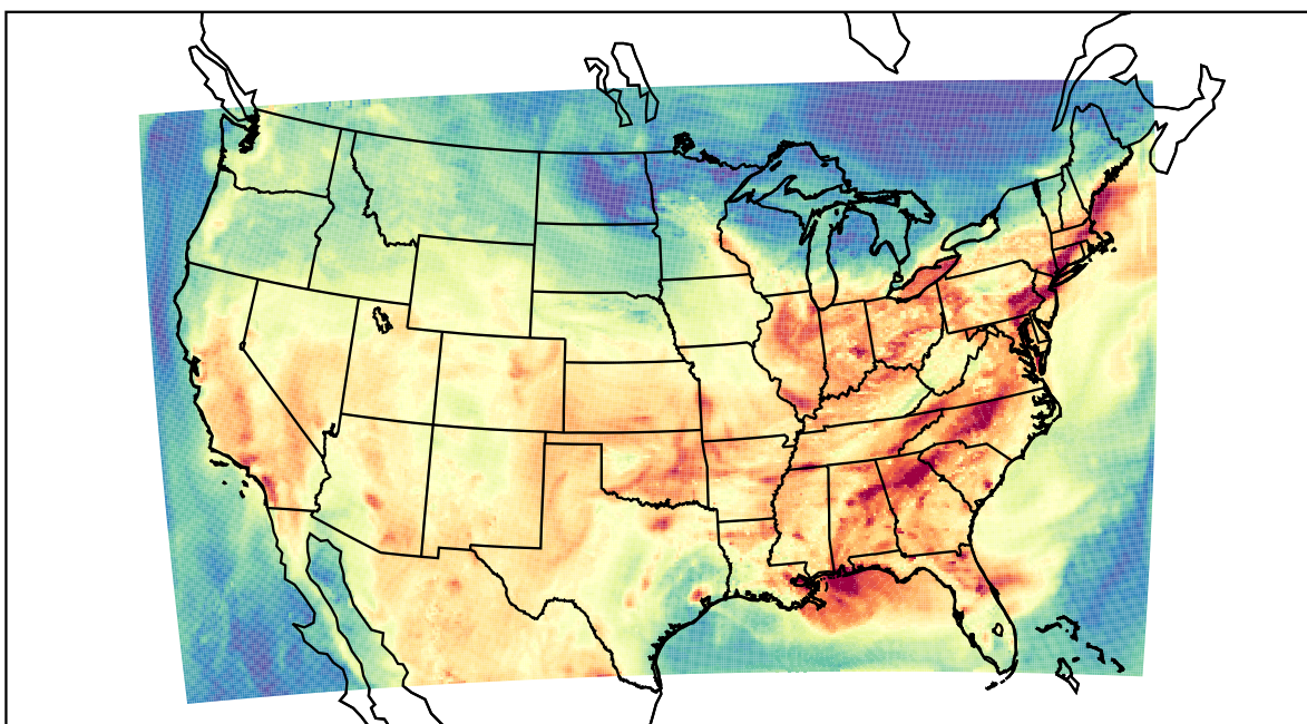
WRF (2019-08-13_20:00:00)
