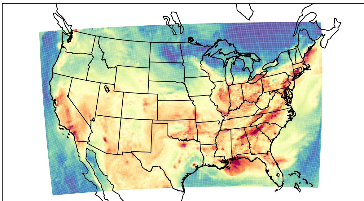
WRF (2019-08-13_22:00:00)
