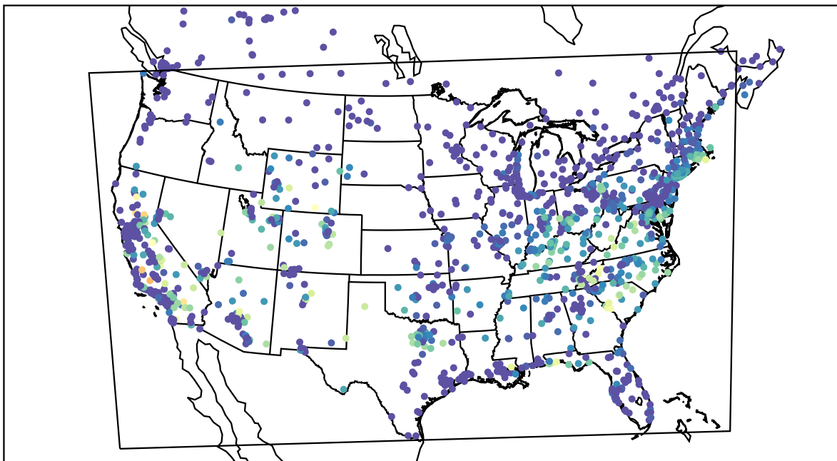
AirNOW (2019-08-14_13:00:00)
