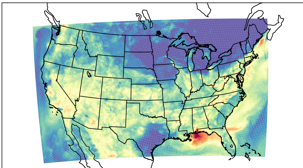
WRF (2019-08-14_06:00:00)
