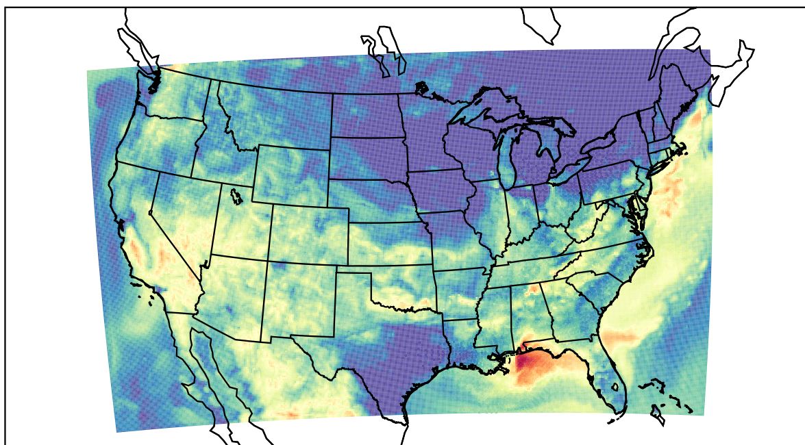
WRF (2019-08-14_10:00:00)
