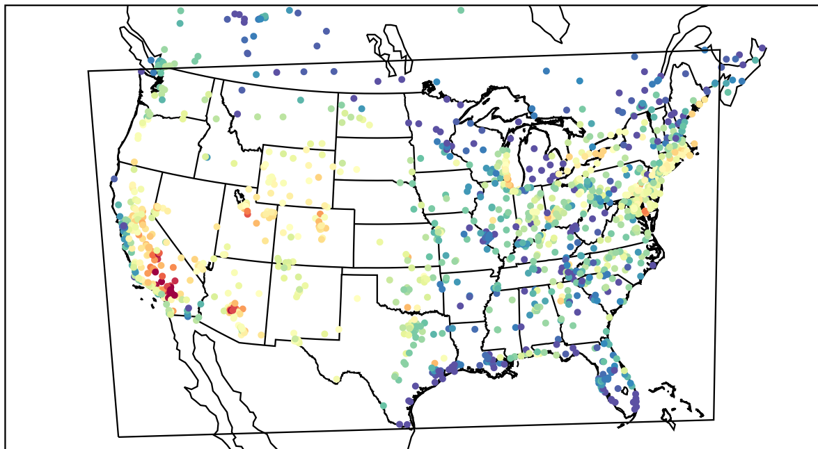
AirNOW (2019-08-13_00:00:00)
