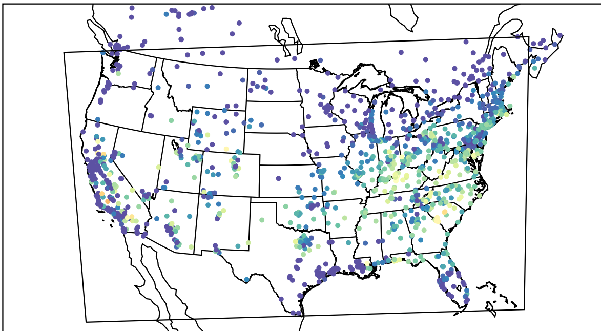
AirNOW (2019-08-14_14:00:00)
