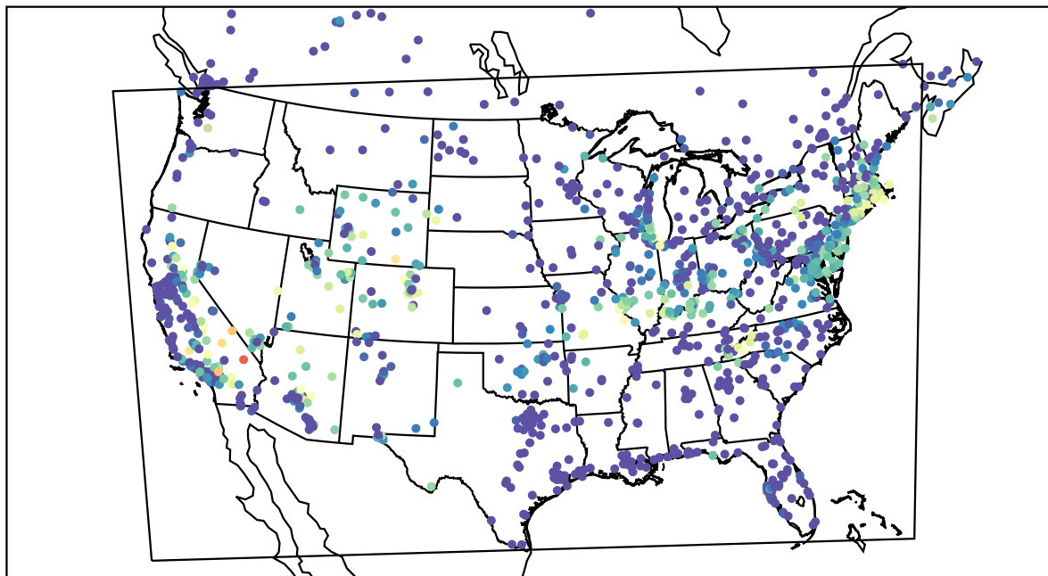
AirNOW (2019-08-13_10:00:00)
