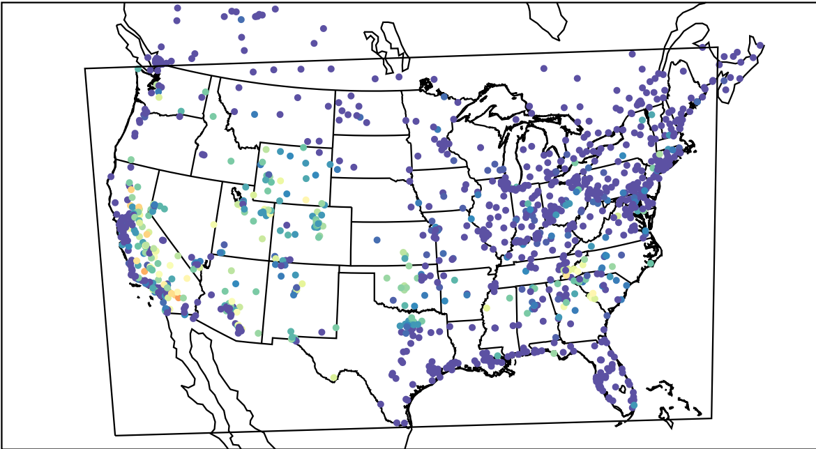
AirNOW (2019-08-14_08:00:00)
