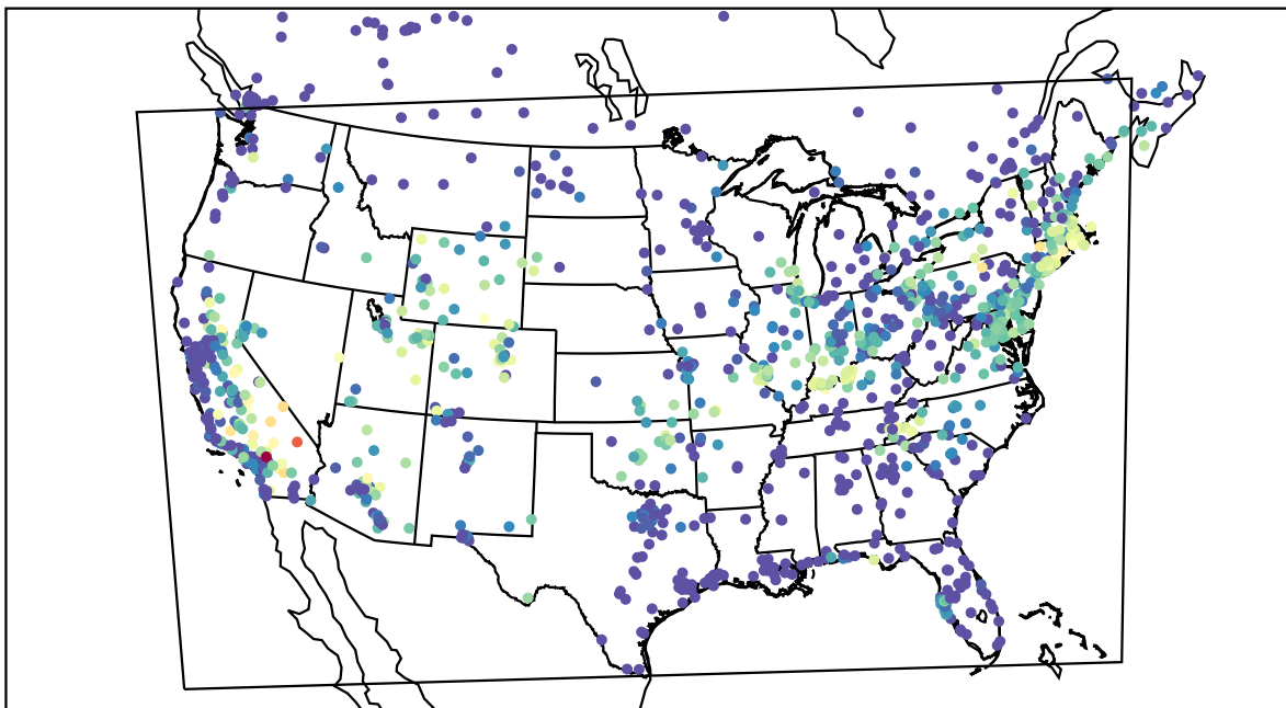
AirNOW (2019-08-13_08:00:00)
