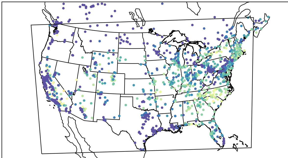
AirNOW (2019-08-13_14:00:00)
