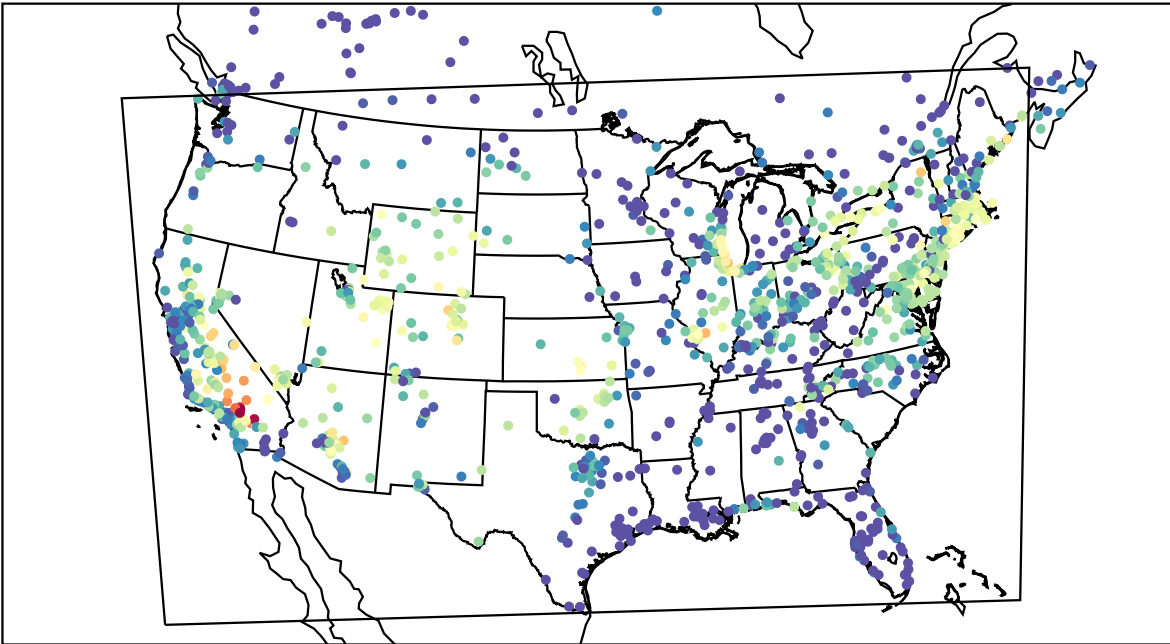
AirNOW (2019-08-13_04:00:00)
