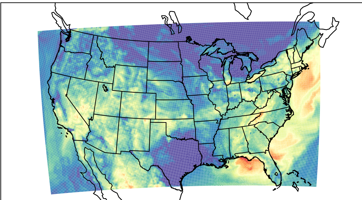
WRF (2019-08-13_13:00:00)
