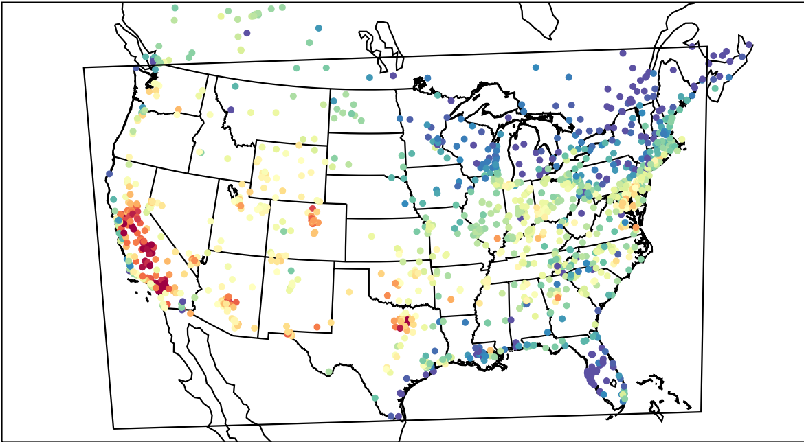
AirNOW (2019-08-14_23:00:00)
