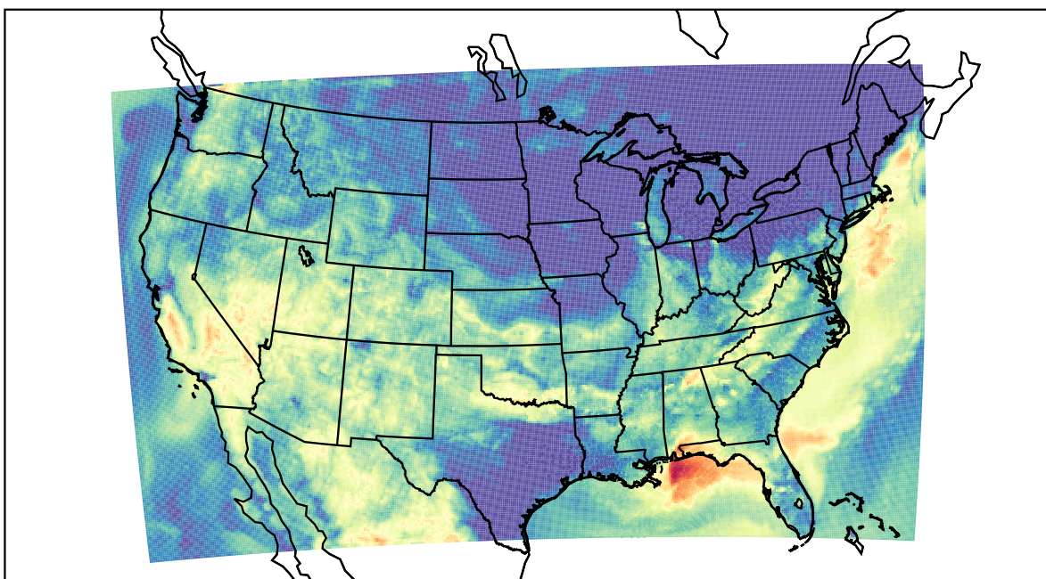
WRF (2019-08-14_11:00:00)
