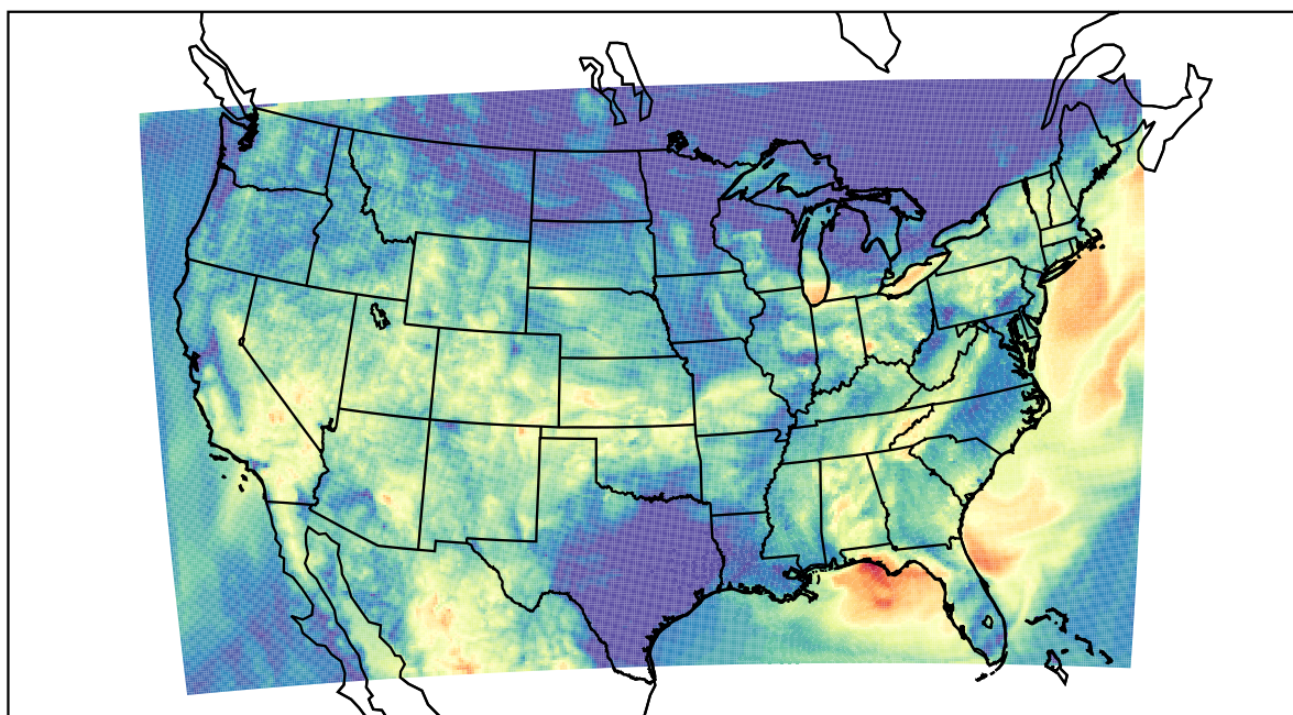
WRF (2019-08-13_10:00:00)
