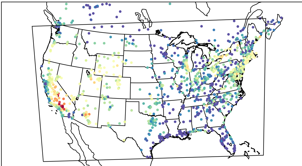
AirNOW (2019-08-13_02:00:00)
