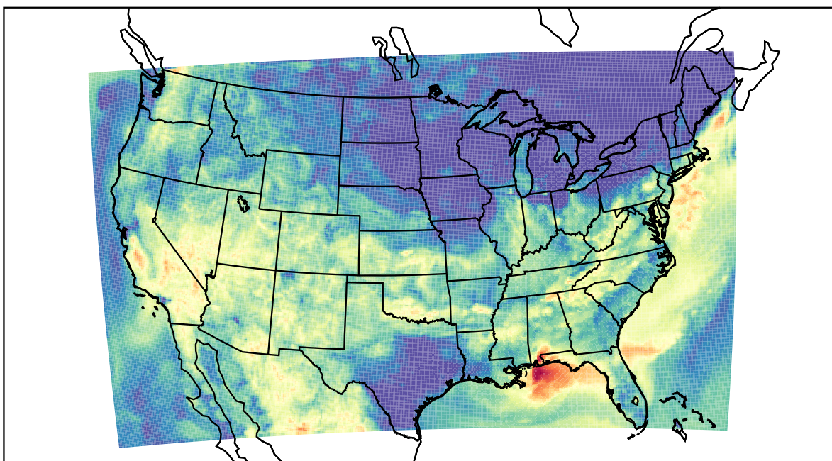
WRF (2019-08-14_09:00:00)
