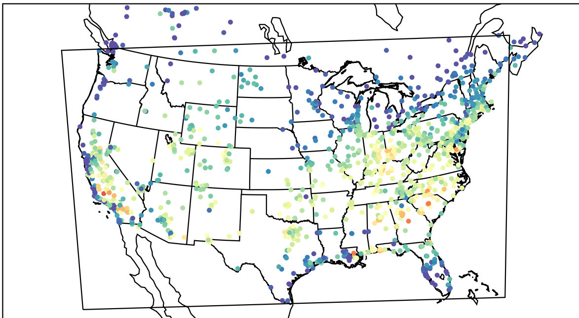
AirNOW (2019-08-14_16:00:00)
