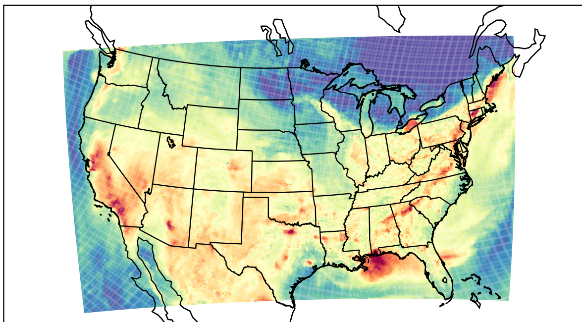
WRF (2019-08-14_00:00:00)
