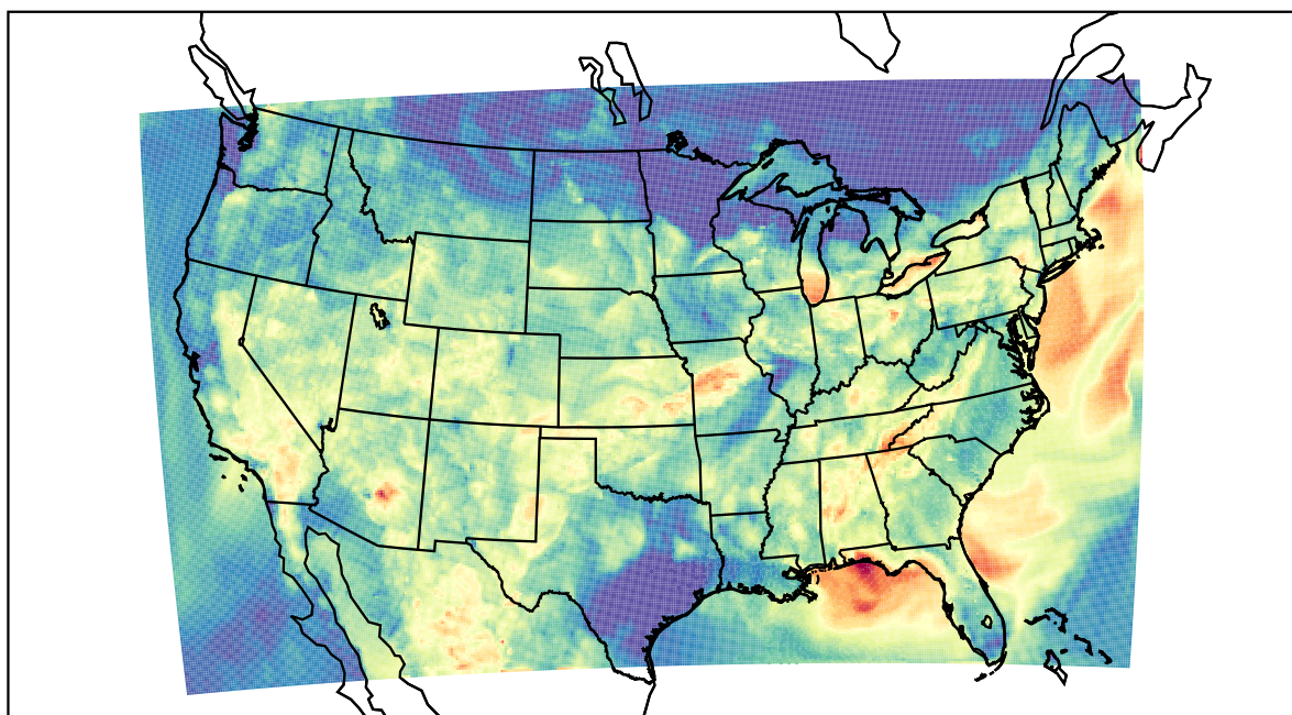
WRF (2019-08-13_05:00:00)
