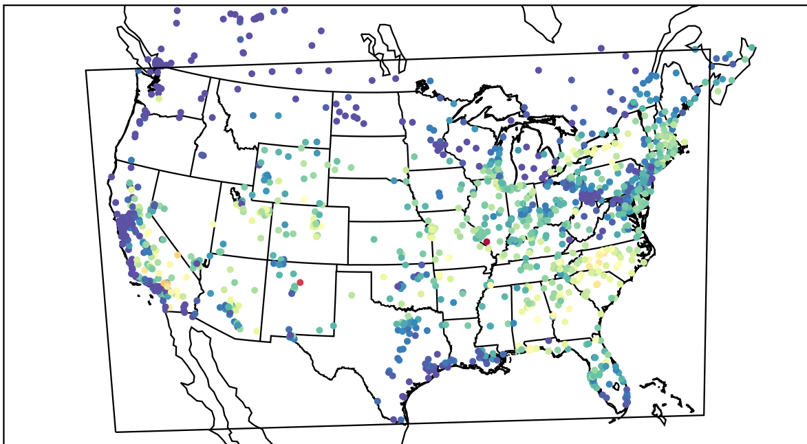
AirNOW (2019-08-13_15:00:00)
