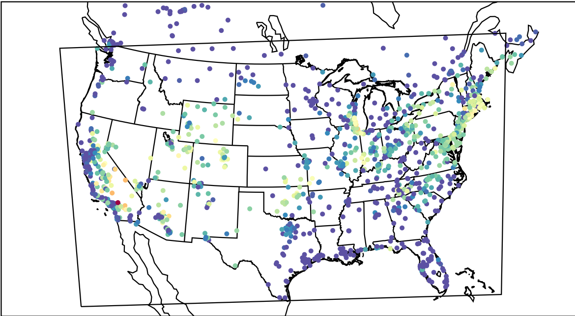
AirNOW (2019-08-13_06:00:00)
