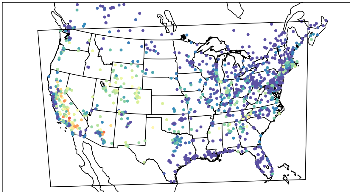
AirNOW (2019-08-14_04:00:00)
