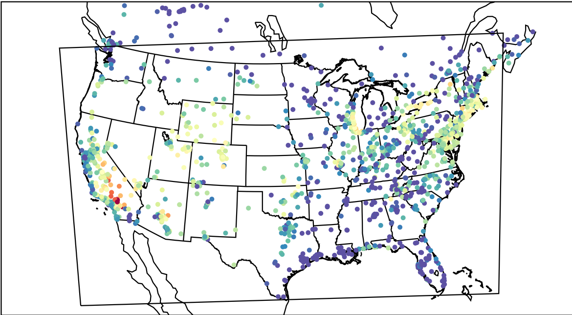
AirNOW (2019-08-13_03:00:00)
