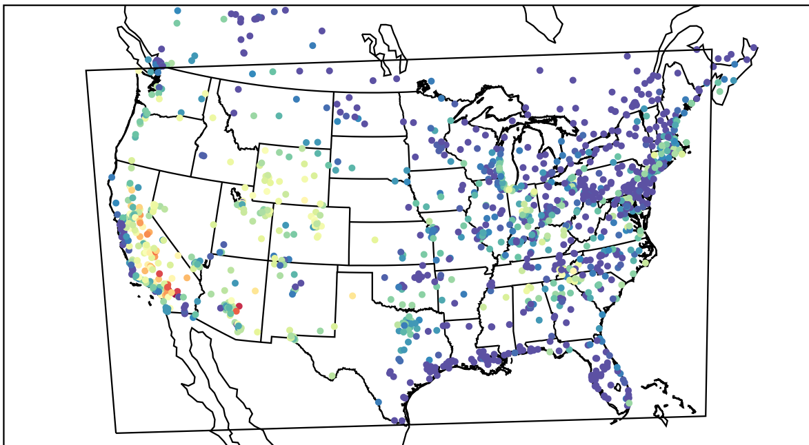
AirNOW (2019-08-14_03:00:00)
