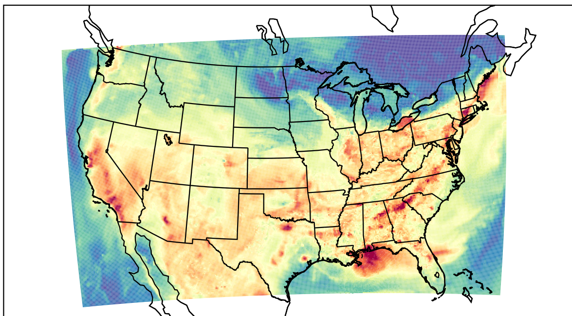
WRF (2019-08-13_23:00:00)
