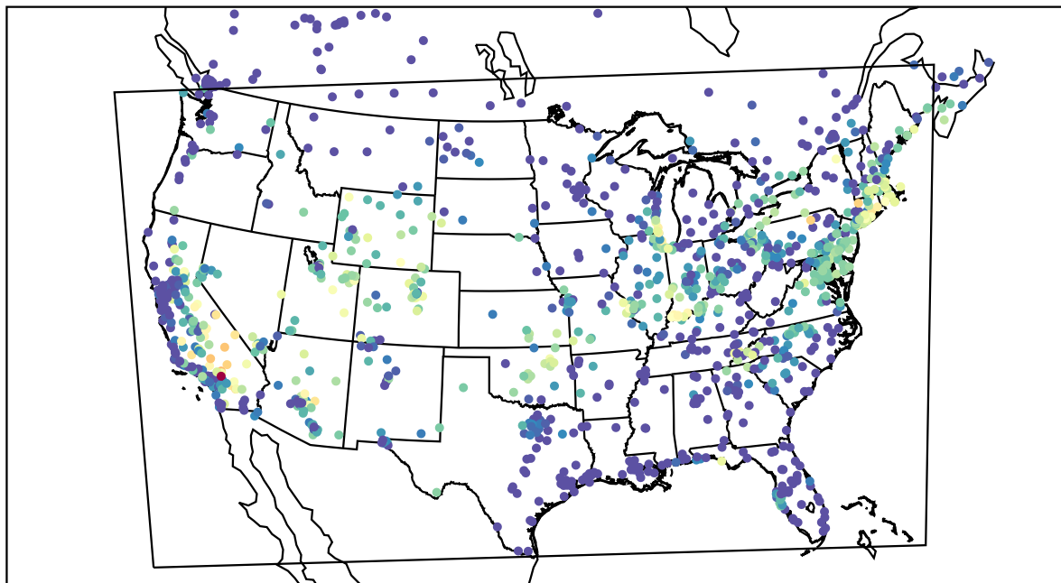
AirNOW (2019-08-13_07:00:00)
