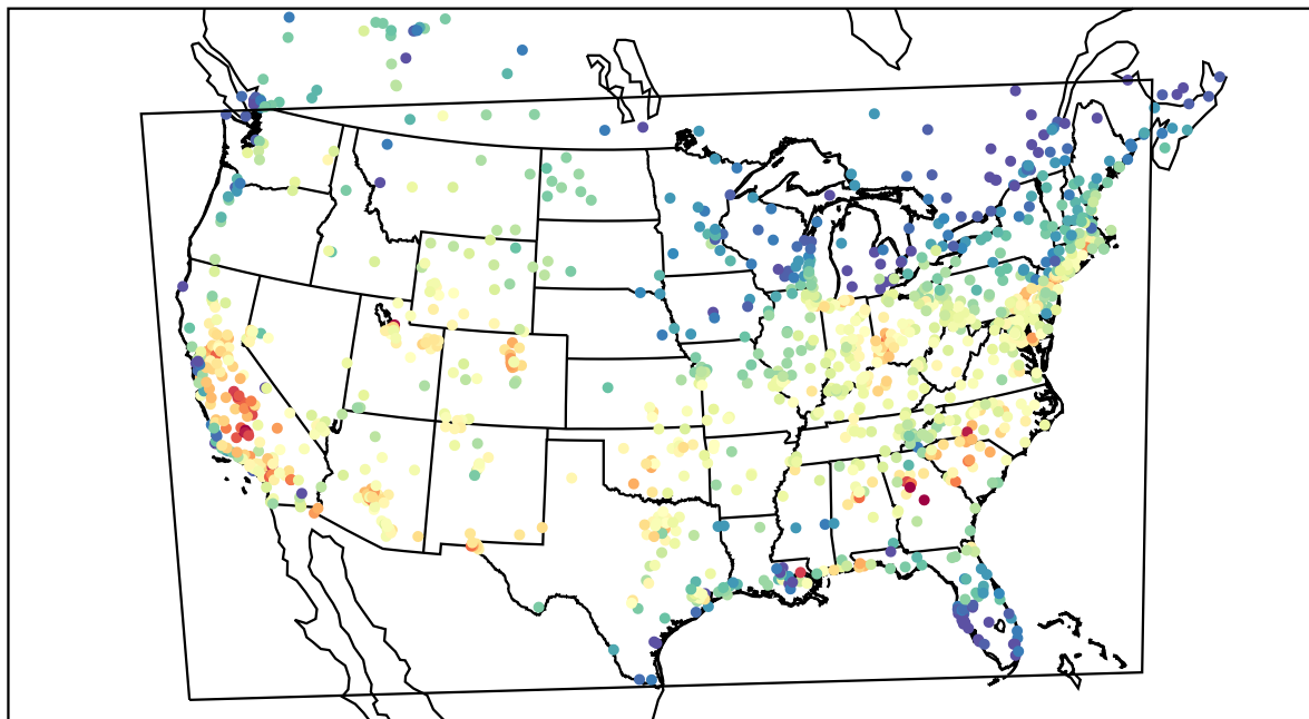
AirNOW (2019-08-14_18:00:00)
