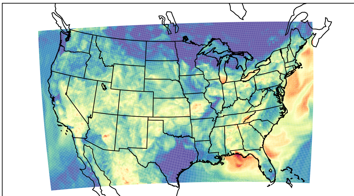
WRF (2019-08-13_07:00:00)
