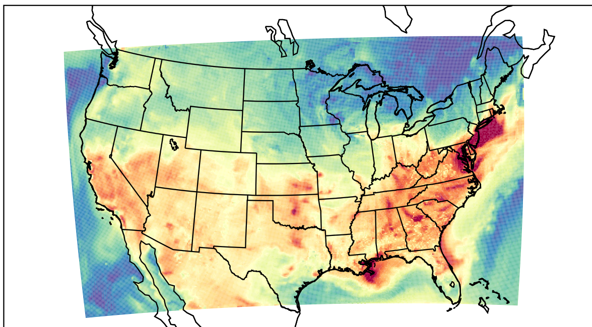
WRF (2019-08-14_19:00:00)
