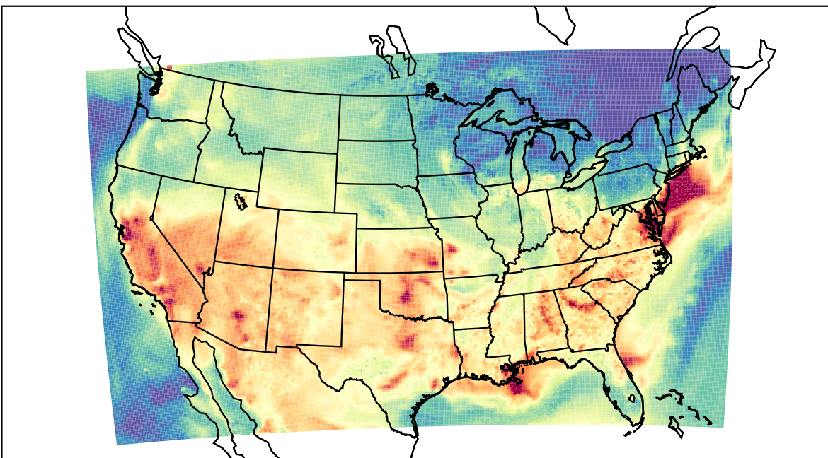
WRF (2019-08-14_23:00:00)
