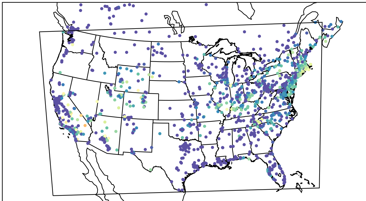
AirNOW (2019-08-13_12:00:00)
