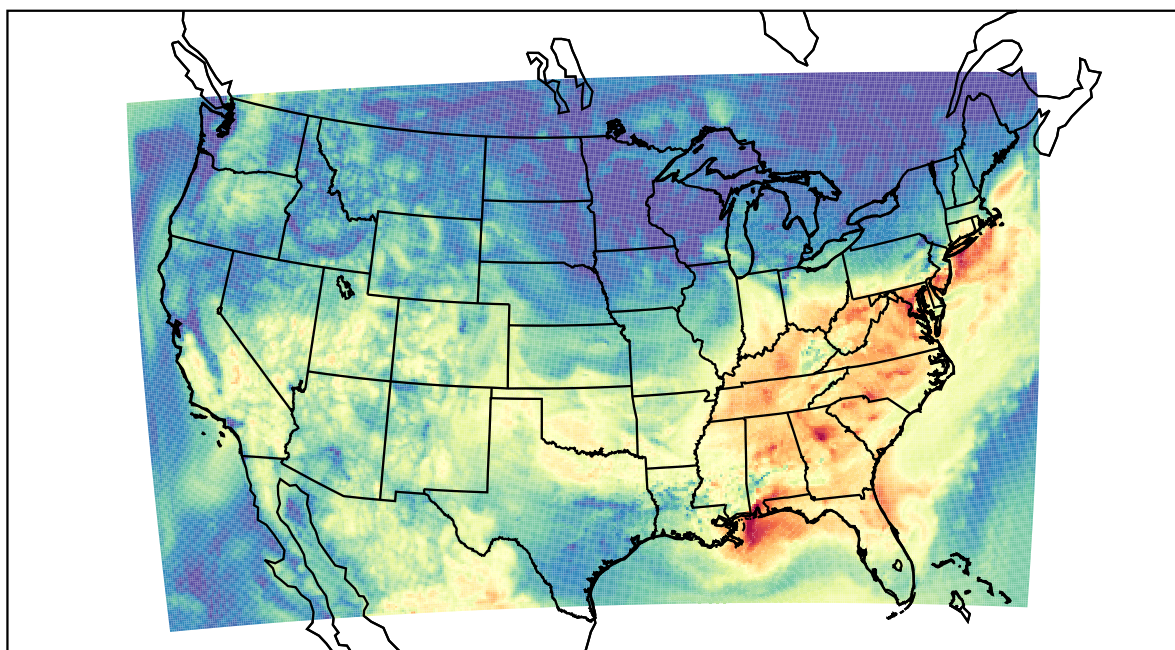
WRF (2019-08-14_15:00:00)
