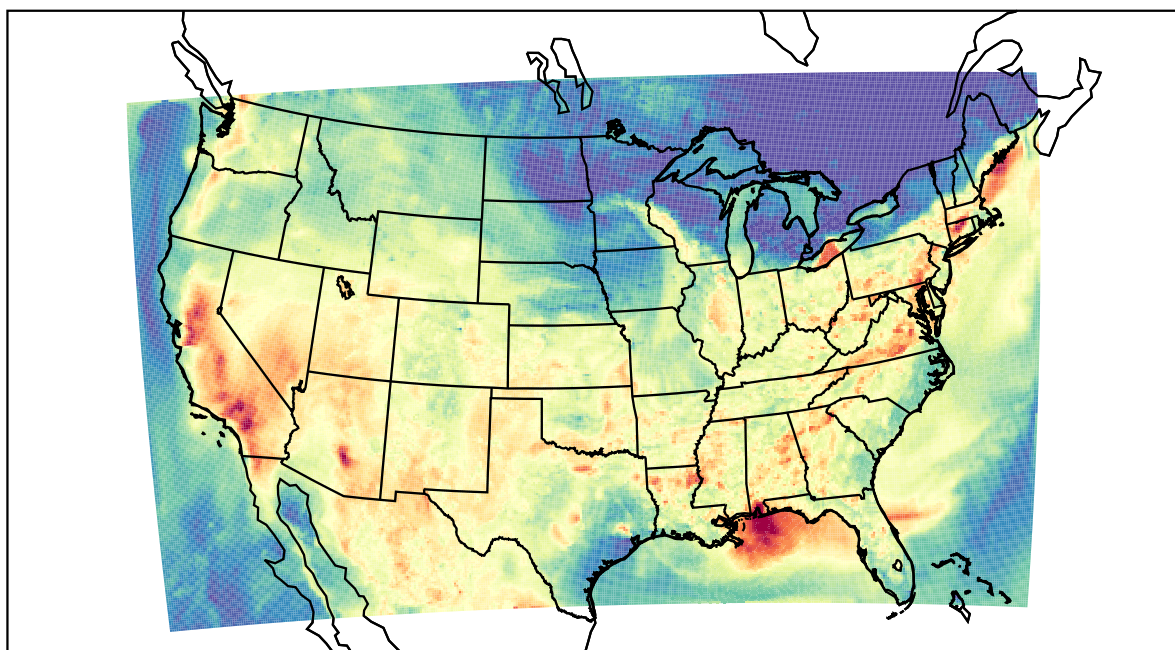
WRF (2019-08-14_01:00:00)
