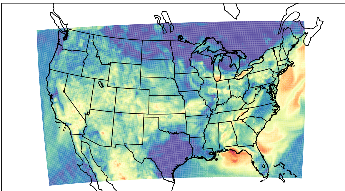
WRF (2019-08-13_09:00:00)
