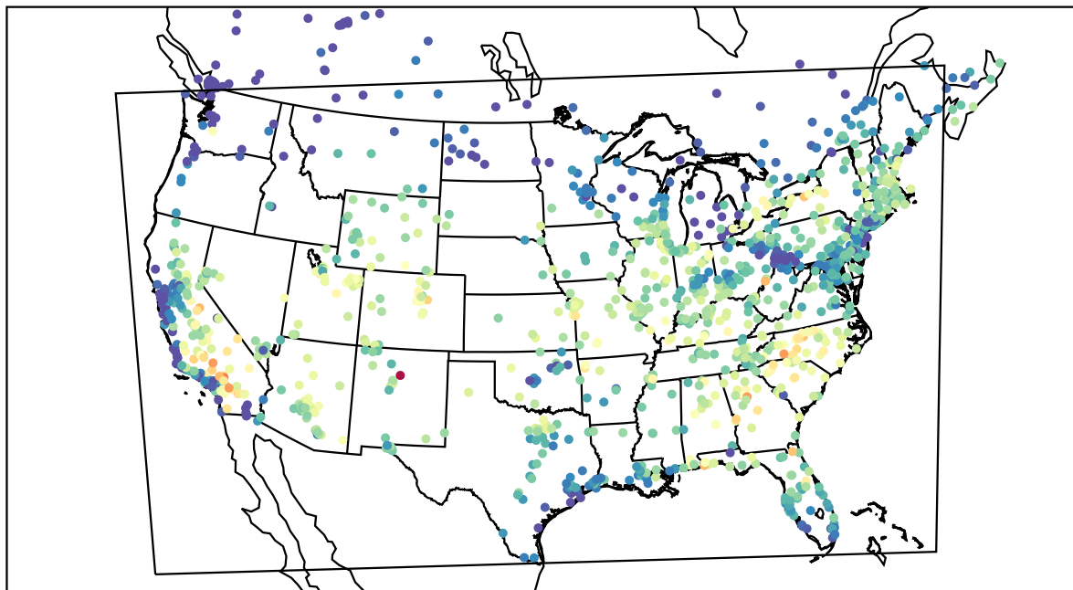
AirNOW (2019-08-13_16:00:00)
