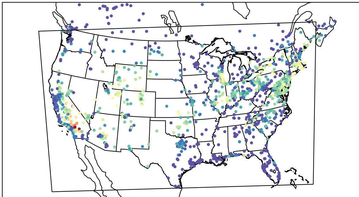
AirNOW (2019-08-13_05:00:00)
