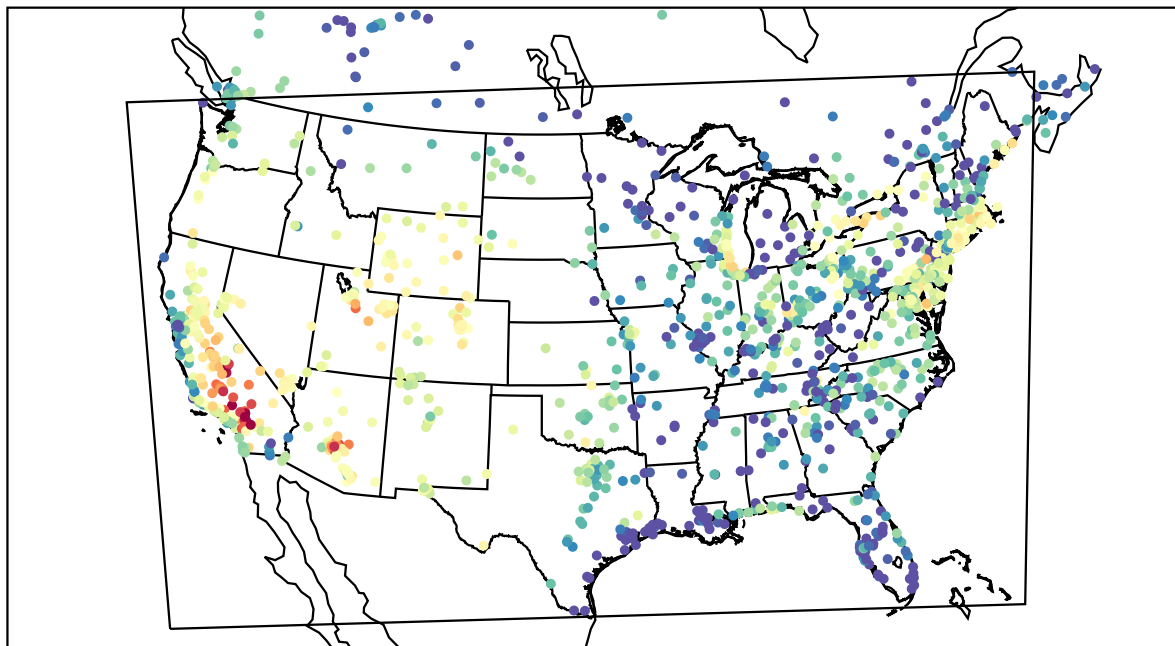
AirNOW (2019-08-13_01:00:00)
