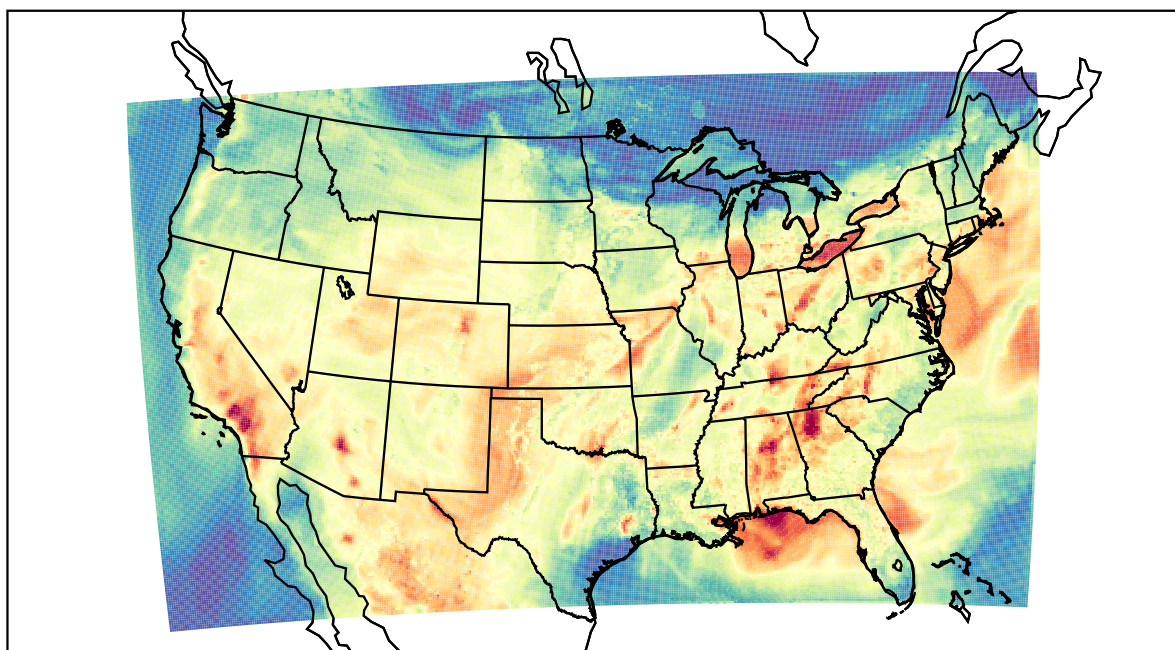
WRF (2019-08-13_00:00:00)
