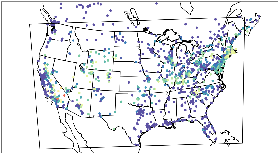
AirNOW (2019-08-13_09:00:00)
