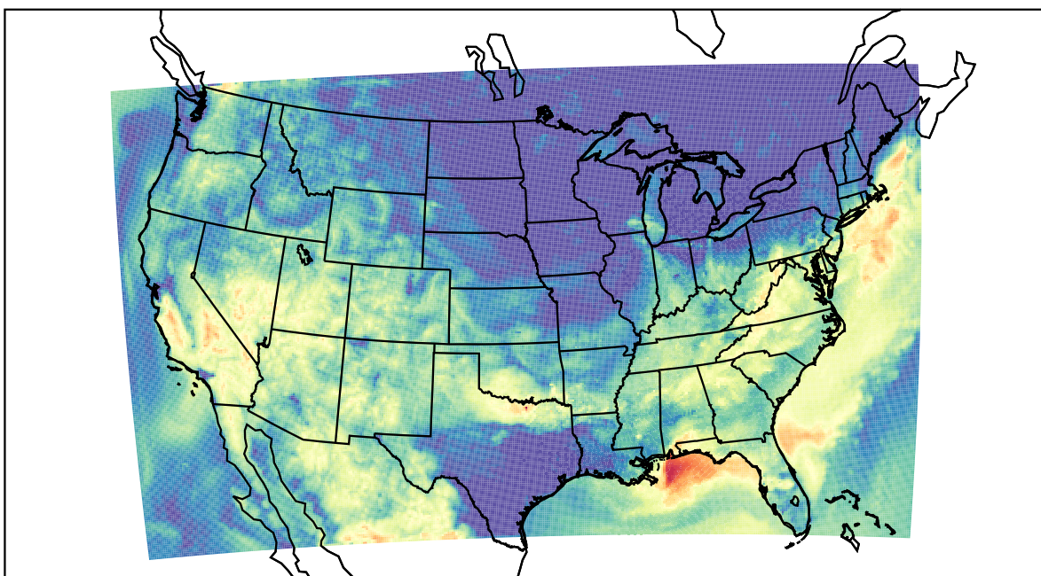
WRF (2019-08-14_13:00:00)
