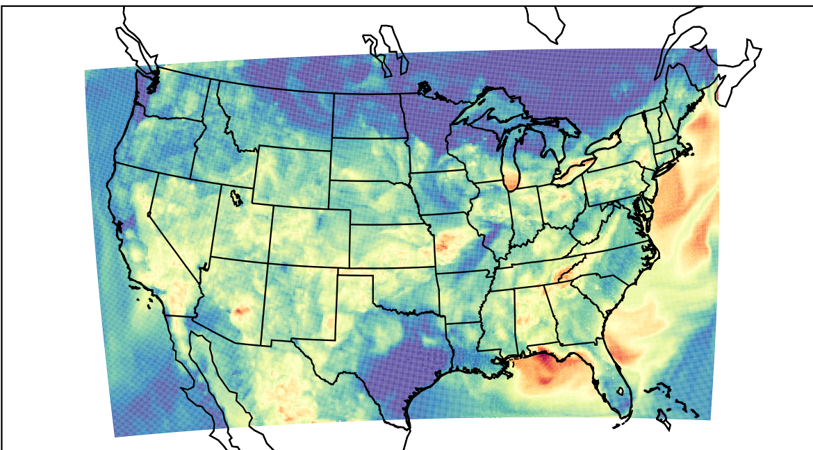
WRF (2019-08-13_06:00:00)
