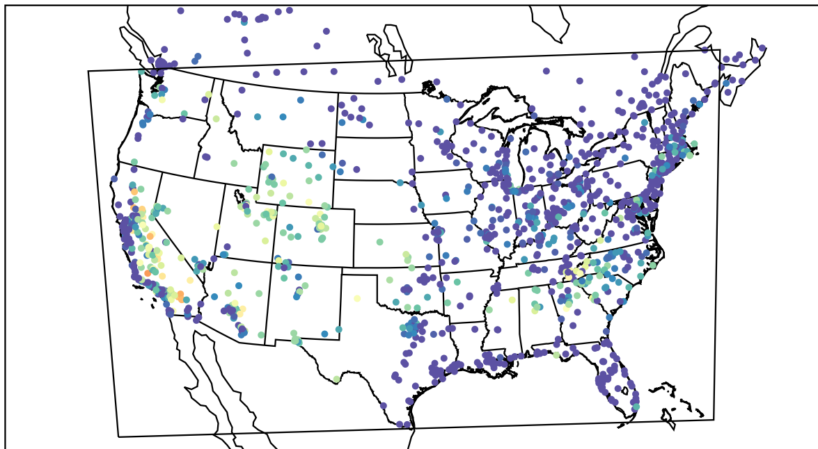
AirNOW (2019-08-14_06:00:00)
