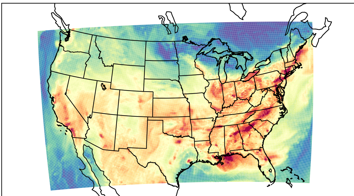
WRF (2019-08-13_21:00:00)
