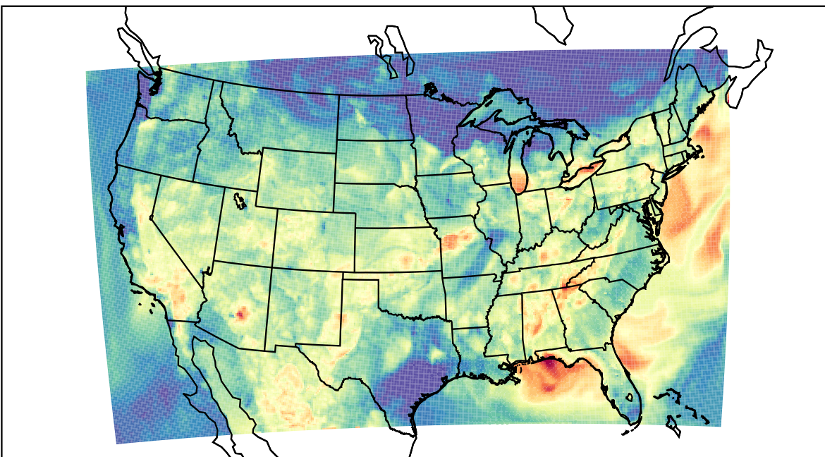
WRF (2019-08-13_04:00:00)
