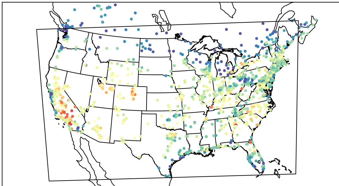
AirNOW (2019-08-13_18:00:00)
