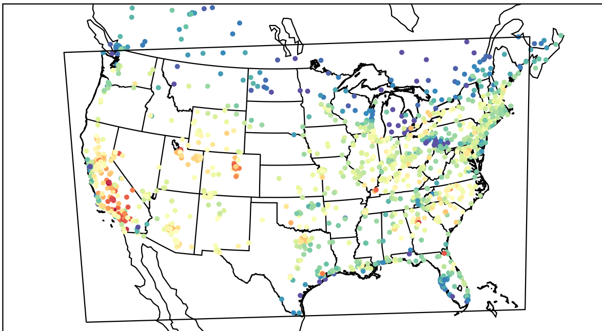
AirNOW (2019-08-13_19:00:00)
