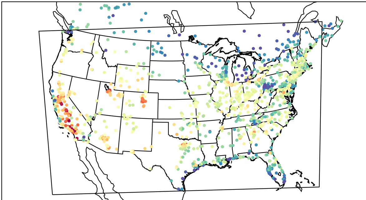
AirNOW (2019-08-13_21:00:00)
