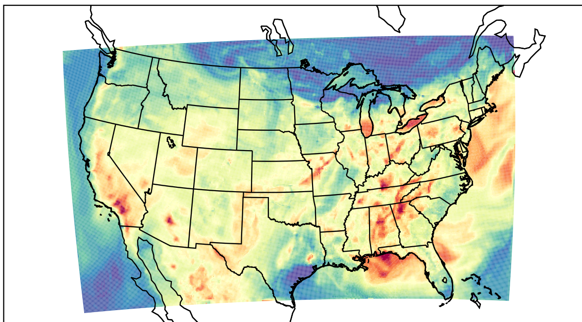
WRF (2019-08-13_01:00:00)
