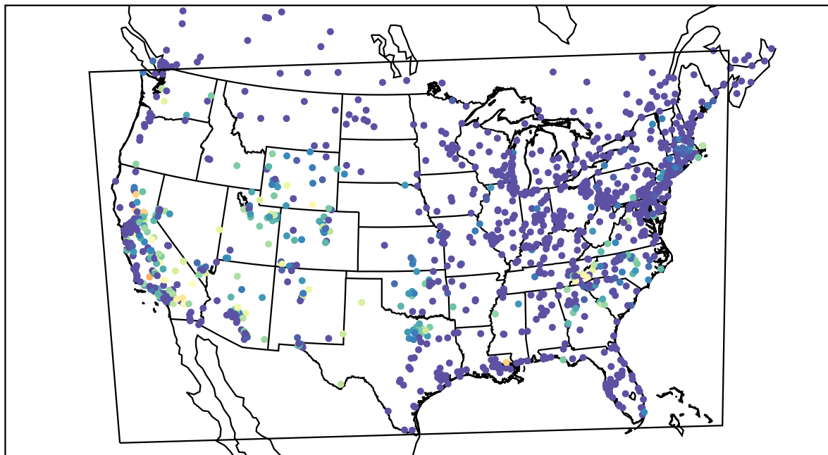
AirNOW (2019-08-14_10:00:00)
