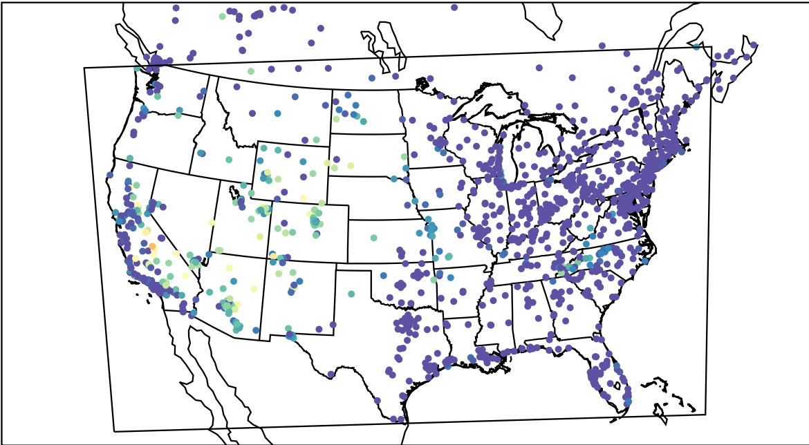
AirNOW (2019-08-24_11:00:00)
