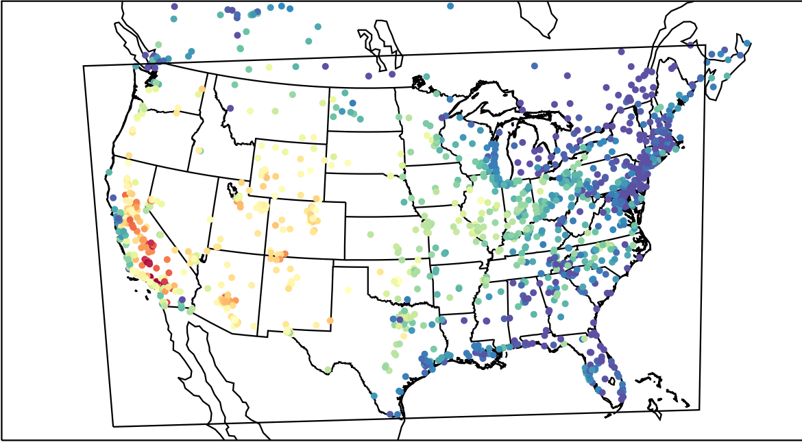
AirNOW (2019-08-23_23:00:00)
