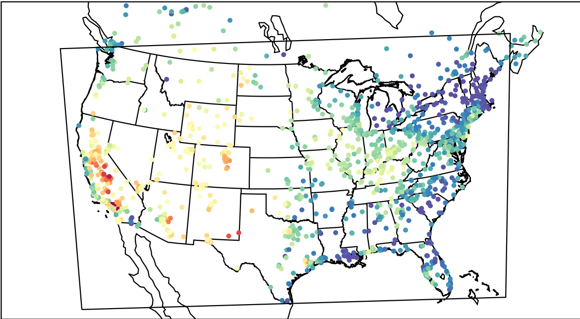
AirNOW (2019-08-24_22:00:00)
