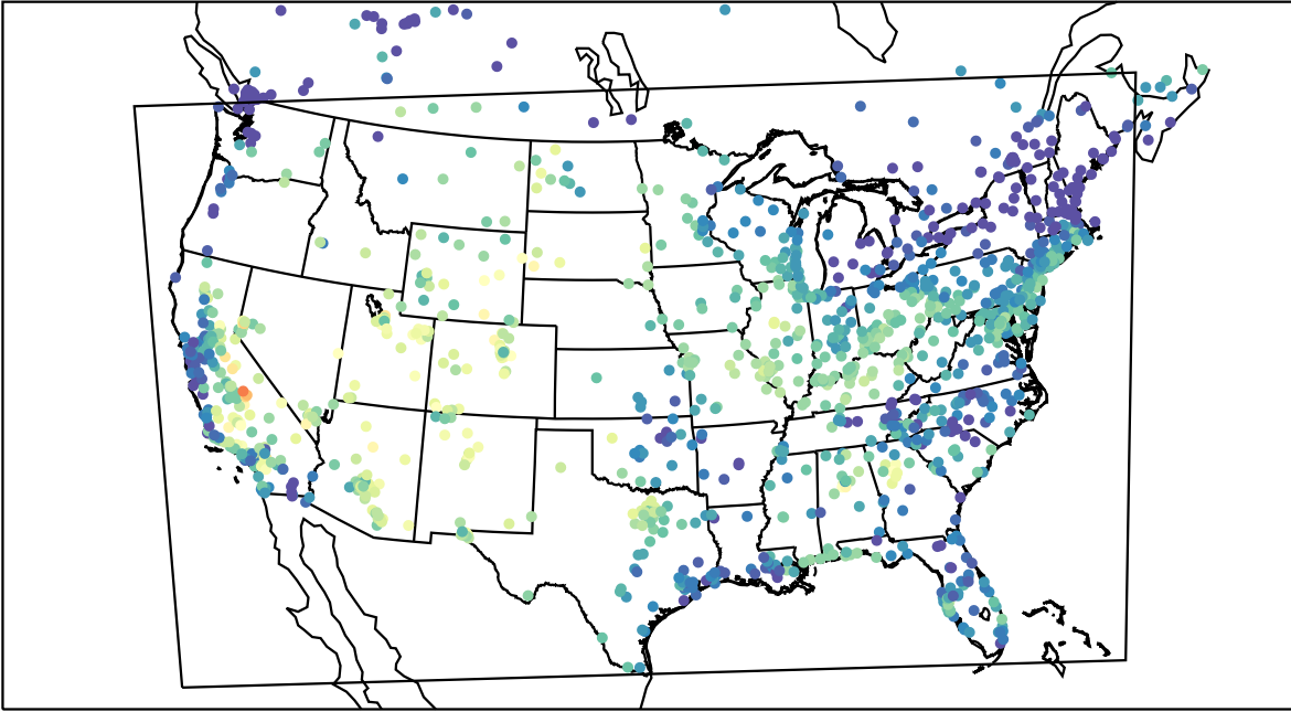
AirNOW (2019-08-24_16:00:00)
