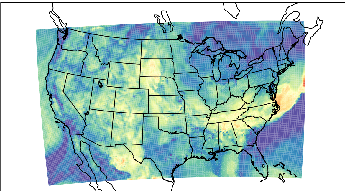
WRF (2019-08-24_15:00:00)
