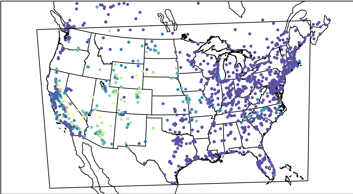
AirNOW (2019-08-24_09:00:00)
