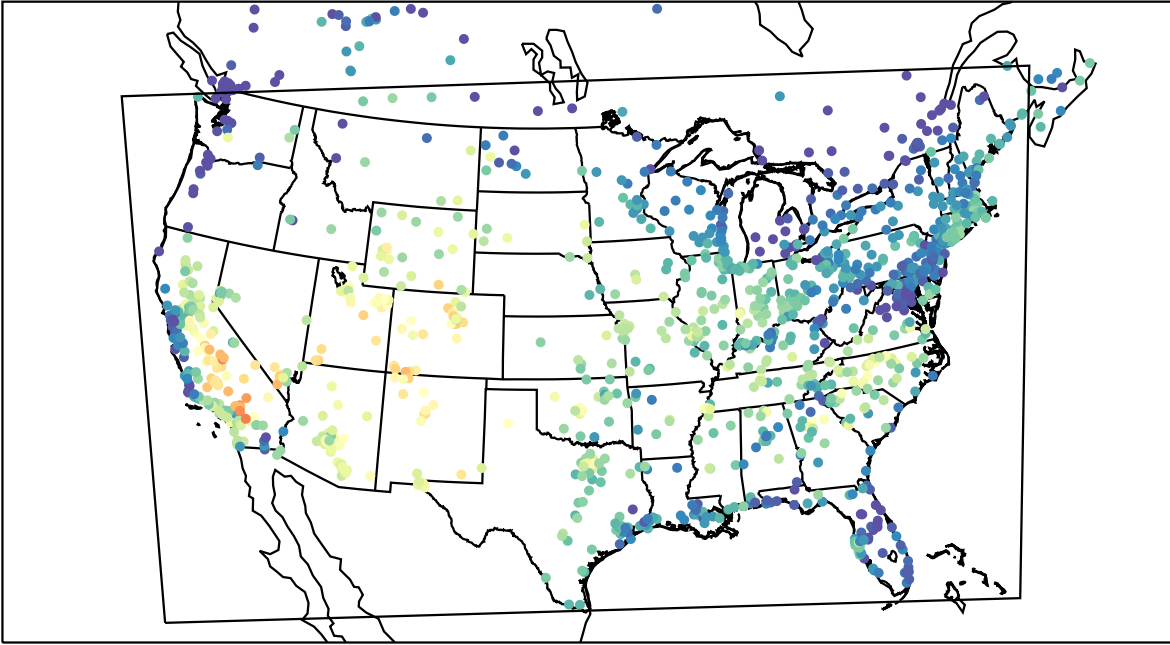
AirNOW (2019-08-23_17:00:00)
