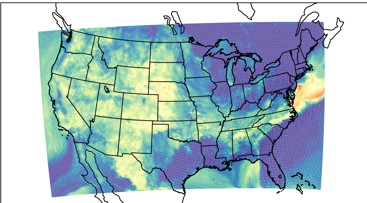
WRF (2019-08-24_06:00:00)
