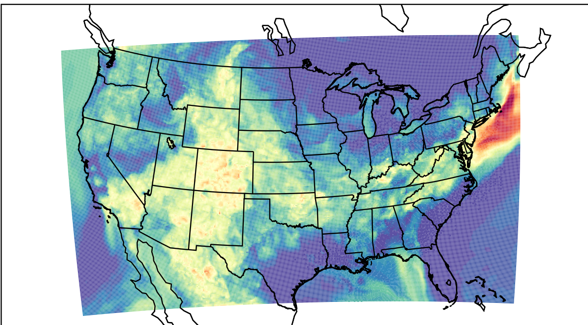
WRF (2019-08-23_06:00:00)
