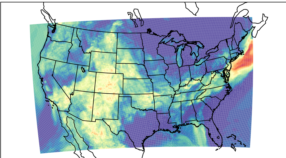
WRF (2019-08-23_08:00:00)
