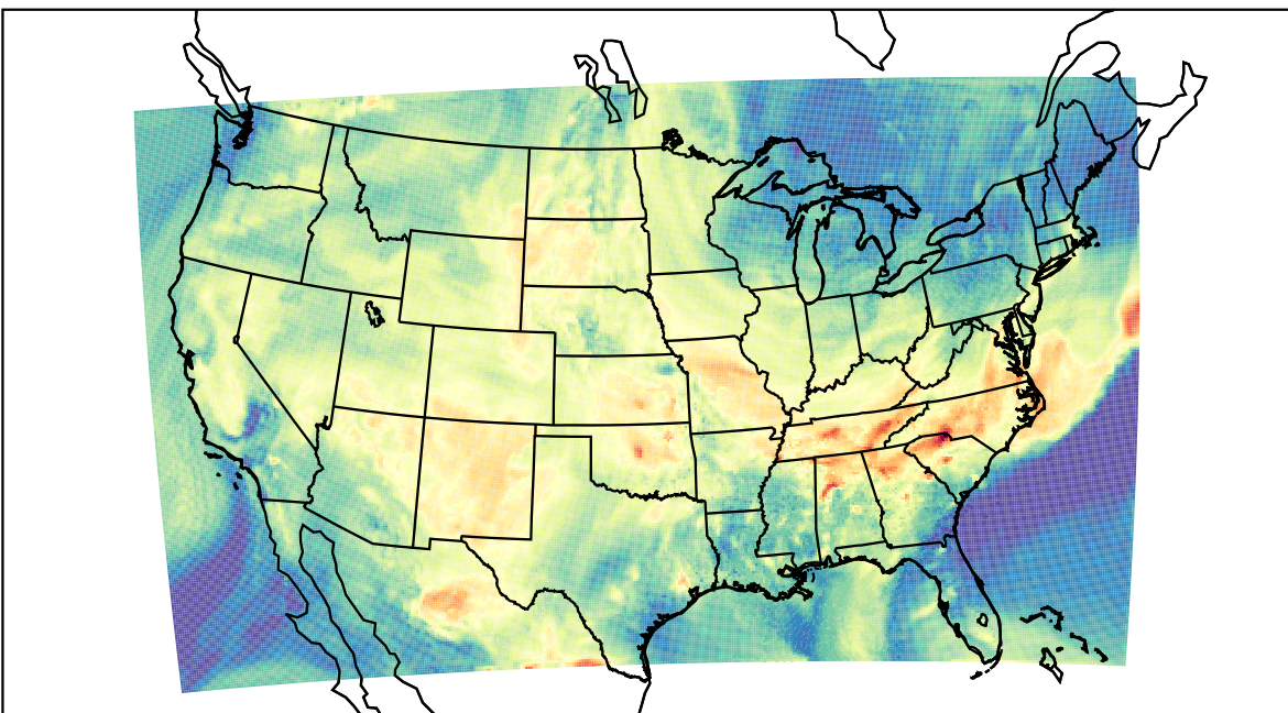
WRF (2019-08-24_18:00:00)
