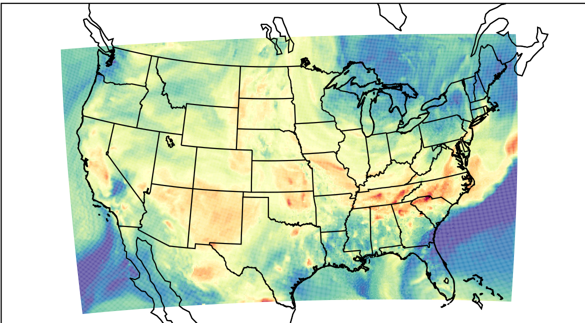
WRF (2019-08-24_20:00:00)
