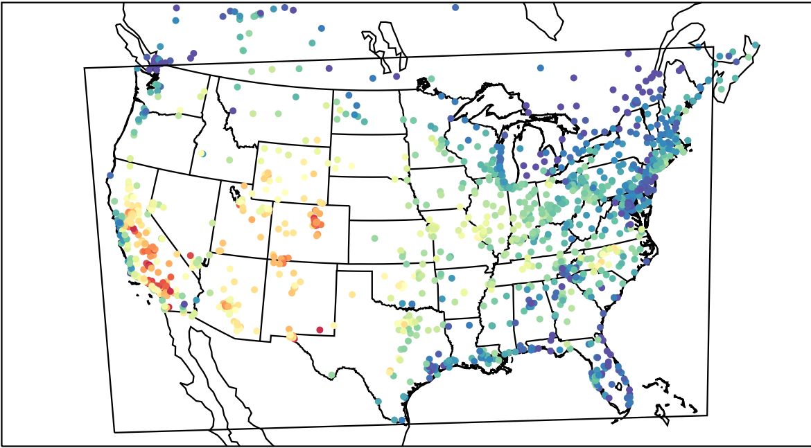
AirNOW (2019-08-23_20:00:00)
