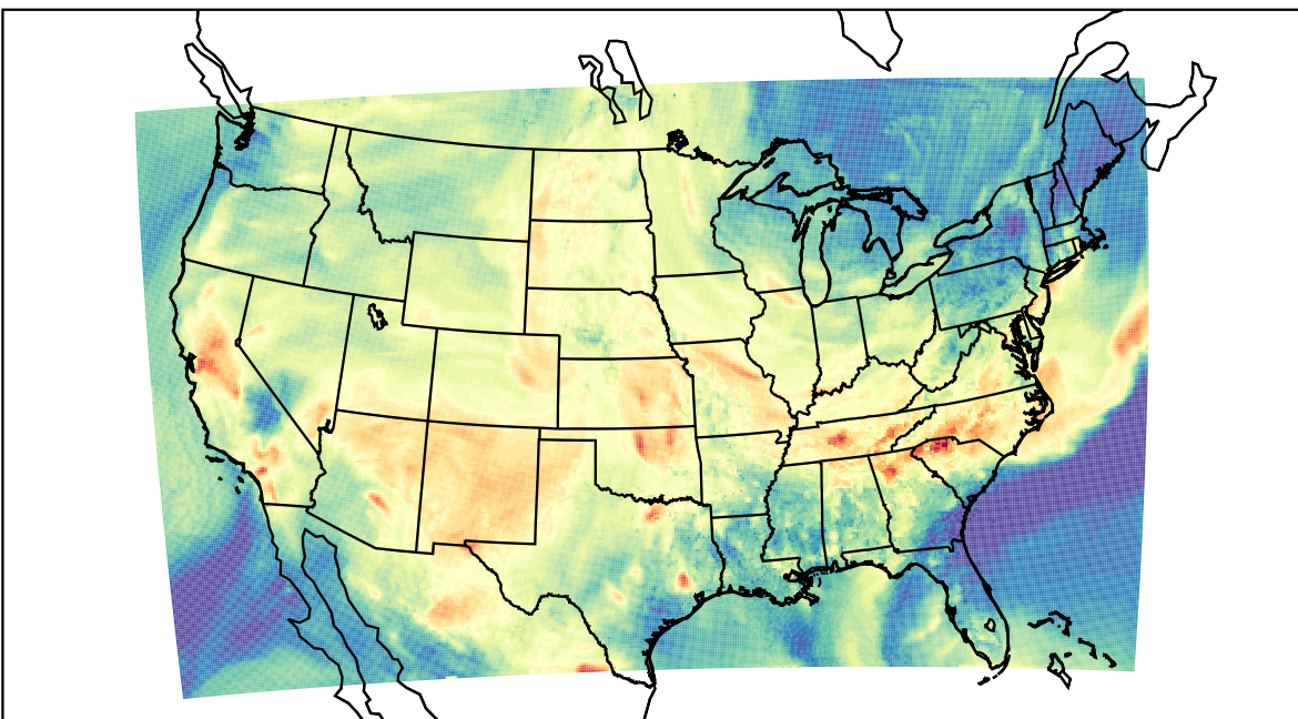
WRF (2019-08-24_22:00:00)
