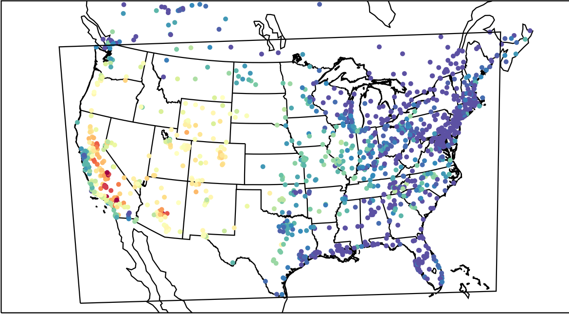
AirNOW (2019-08-24_01:00:00)
