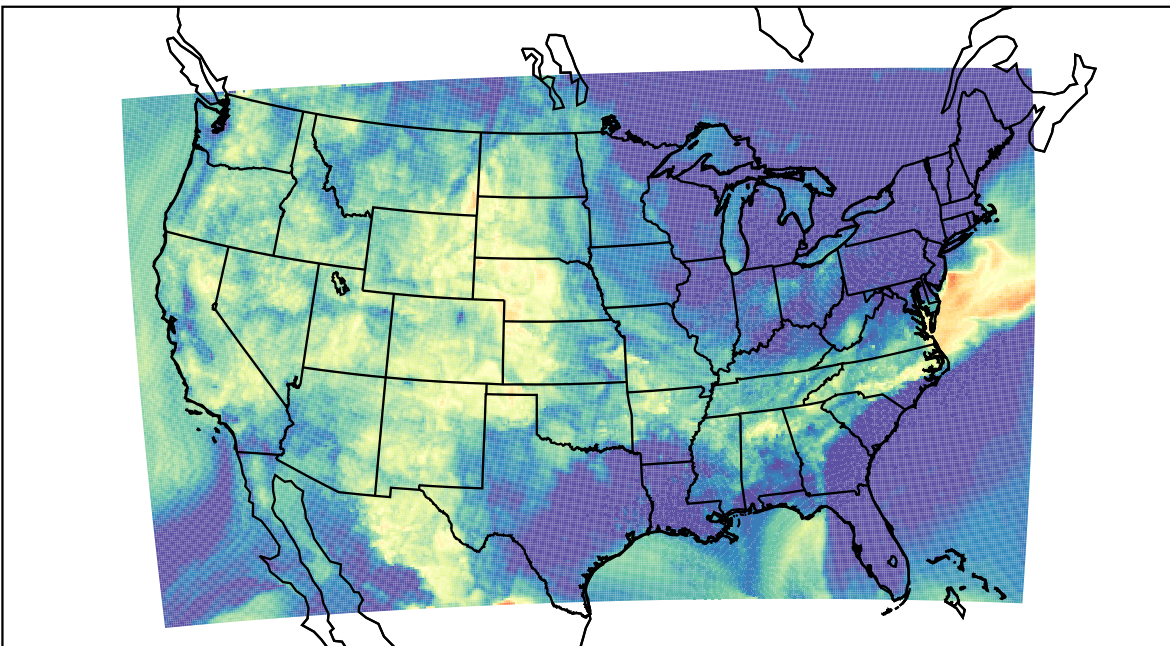
WRF (2019-08-24_07:00:00)
