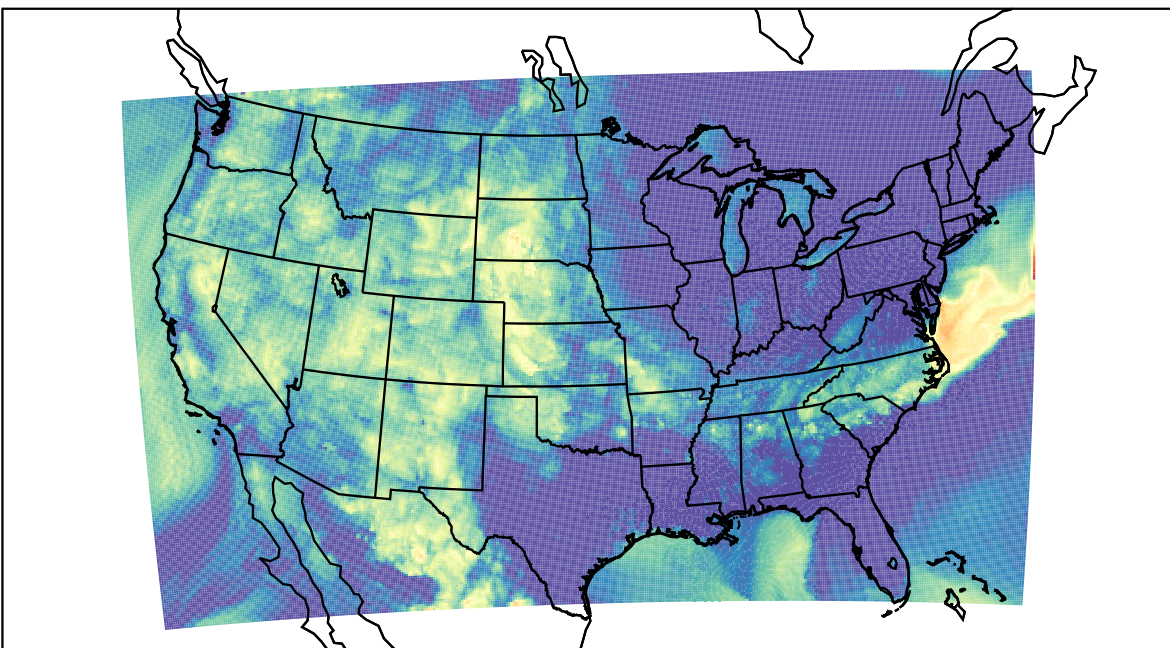
WRF (2019-08-24_12:00:00)
