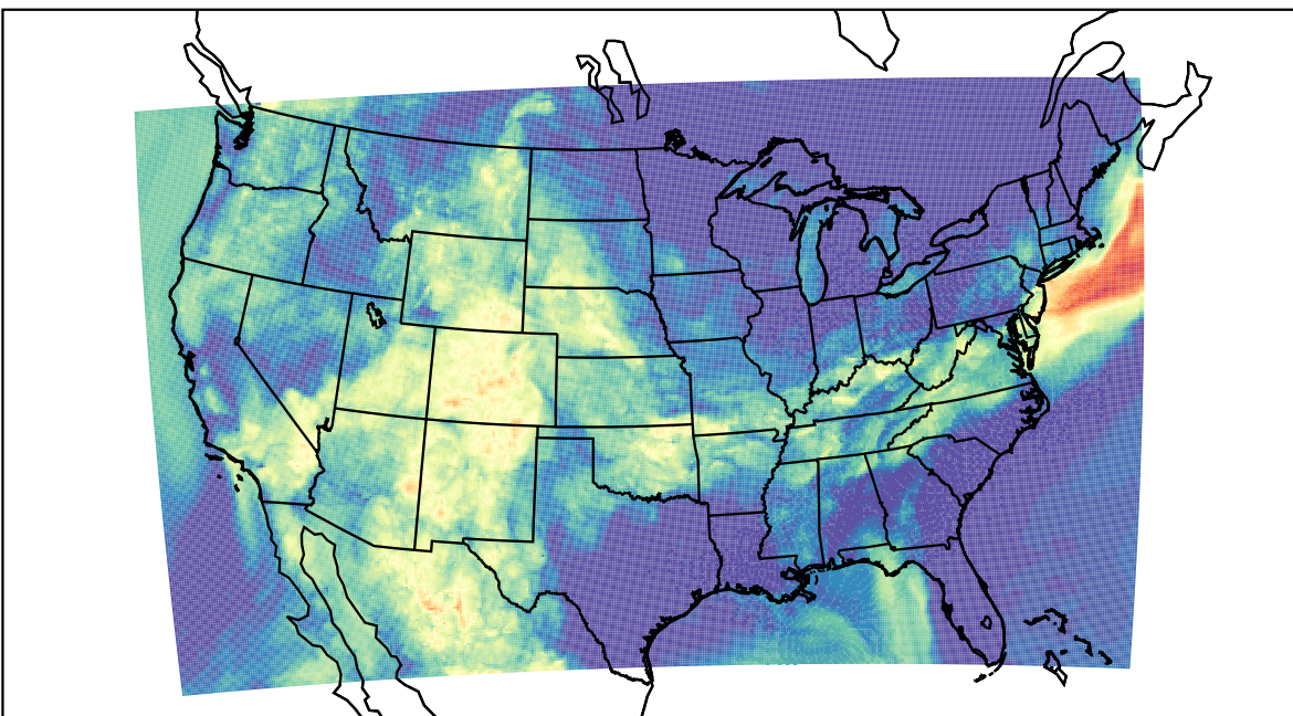
WRF (2019-08-23_09:00:00)
