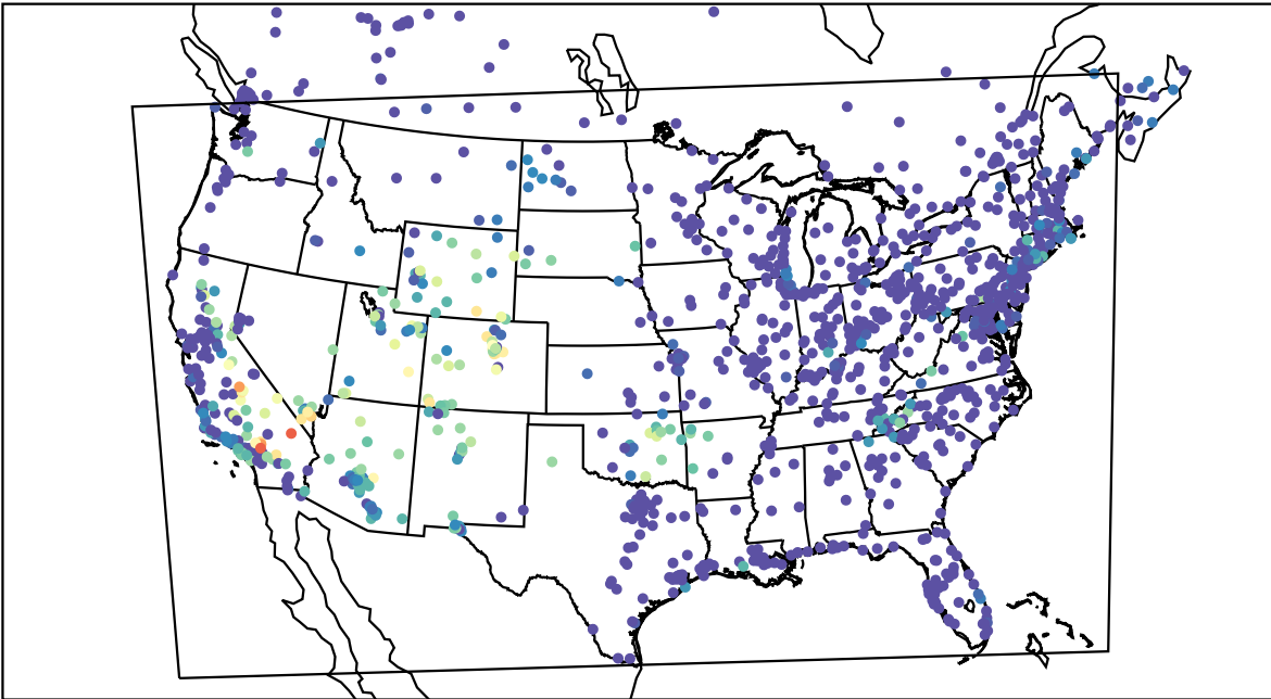
AirNOW (2019-08-23_11:00:00)
