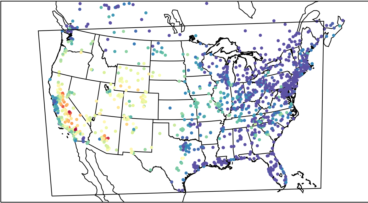
AirNOW (2019-08-24_02:00:00)
