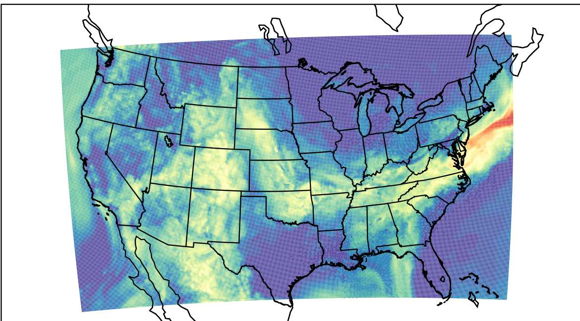
WRF (2019-08-23_14:00:00)
