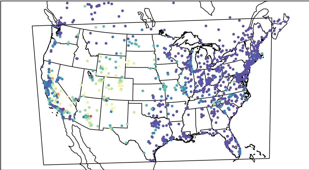
AirNOW (2019-08-24_06:00:00)
