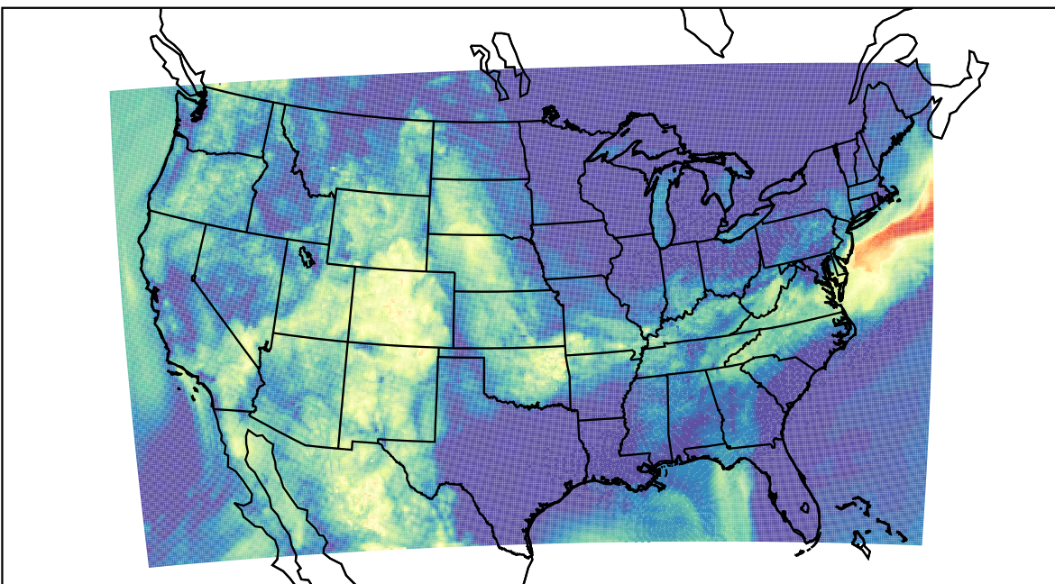
WRF (2019-08-23_13:00:00)
