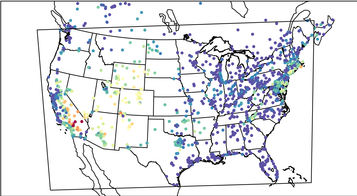
AirNOW (2019-08-23_04:00:00)
