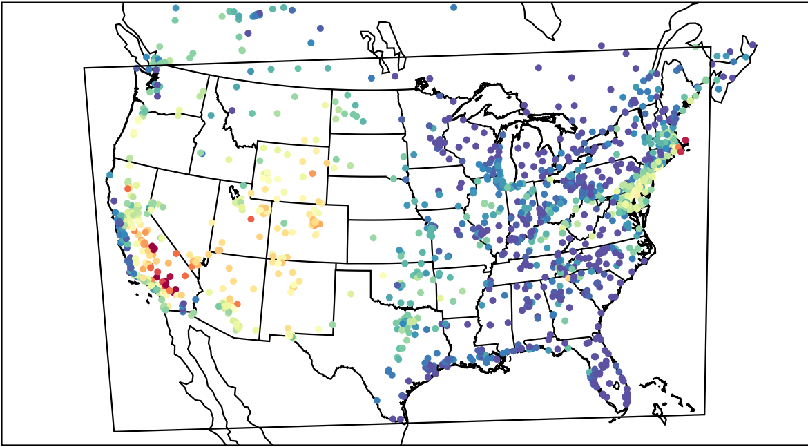
AirNOW (2019-08-23_01:00:00)
