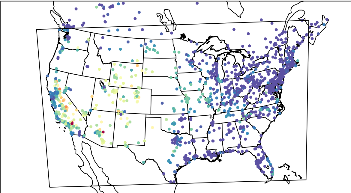
AirNOW (2019-08-24_04:00:00)
