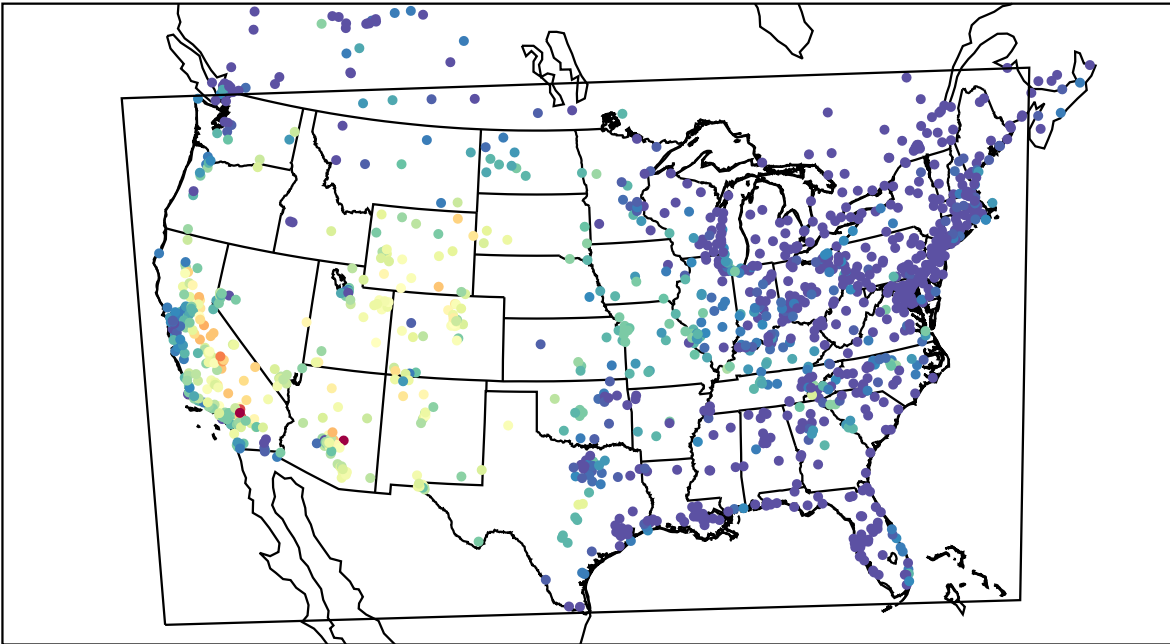
AirNOW (2019-08-24_03:00:00)
