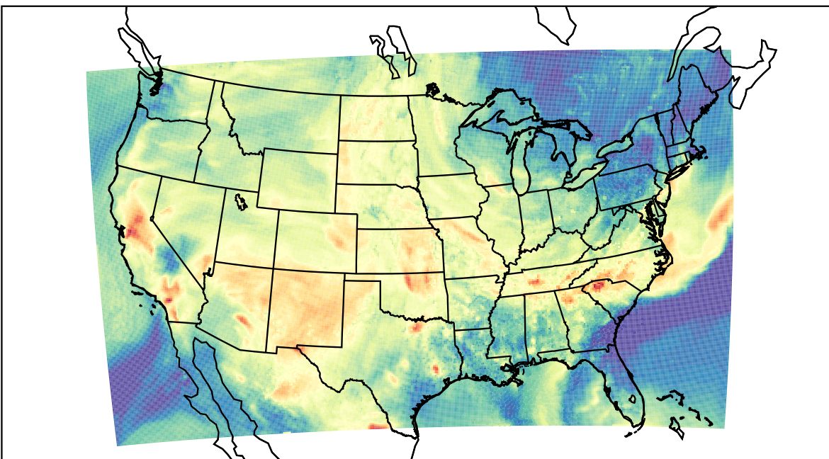
WRF (2019-08-24_23:00:00)
