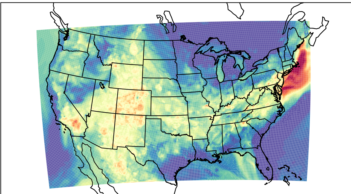
WRF (2019-08-23_03:00:00)
