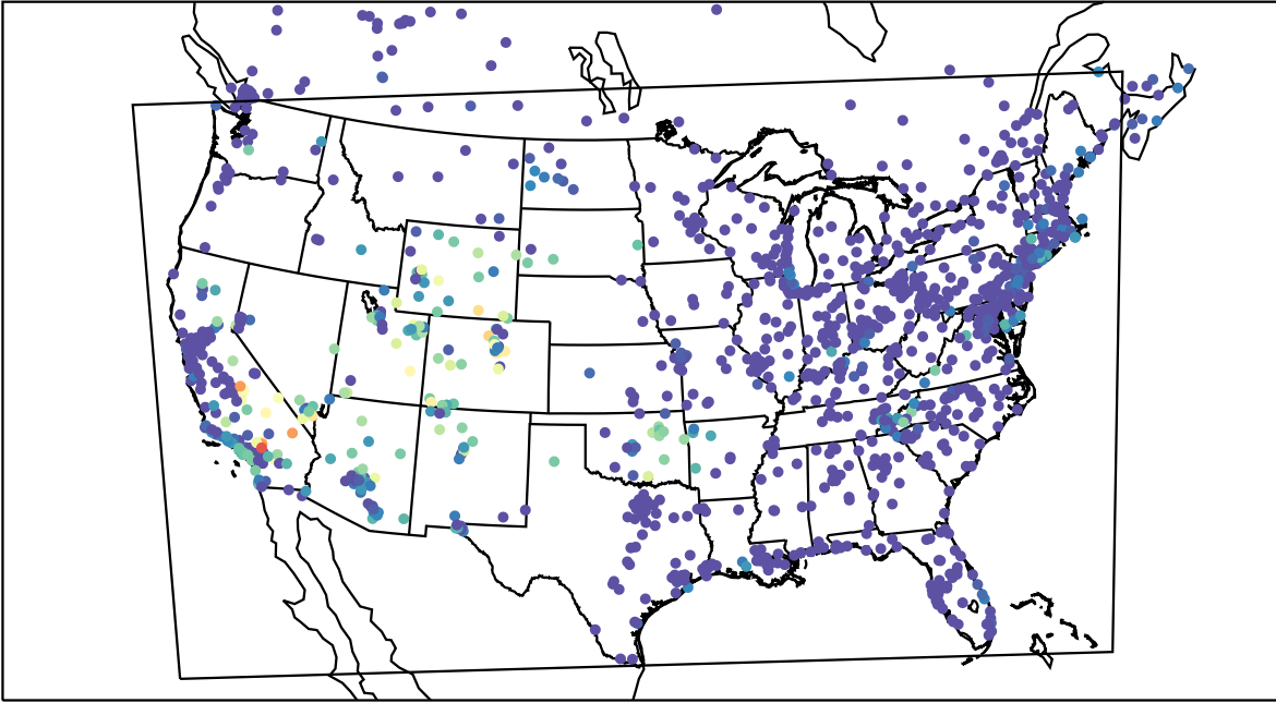
AirNOW (2019-08-23_12:00:00)
