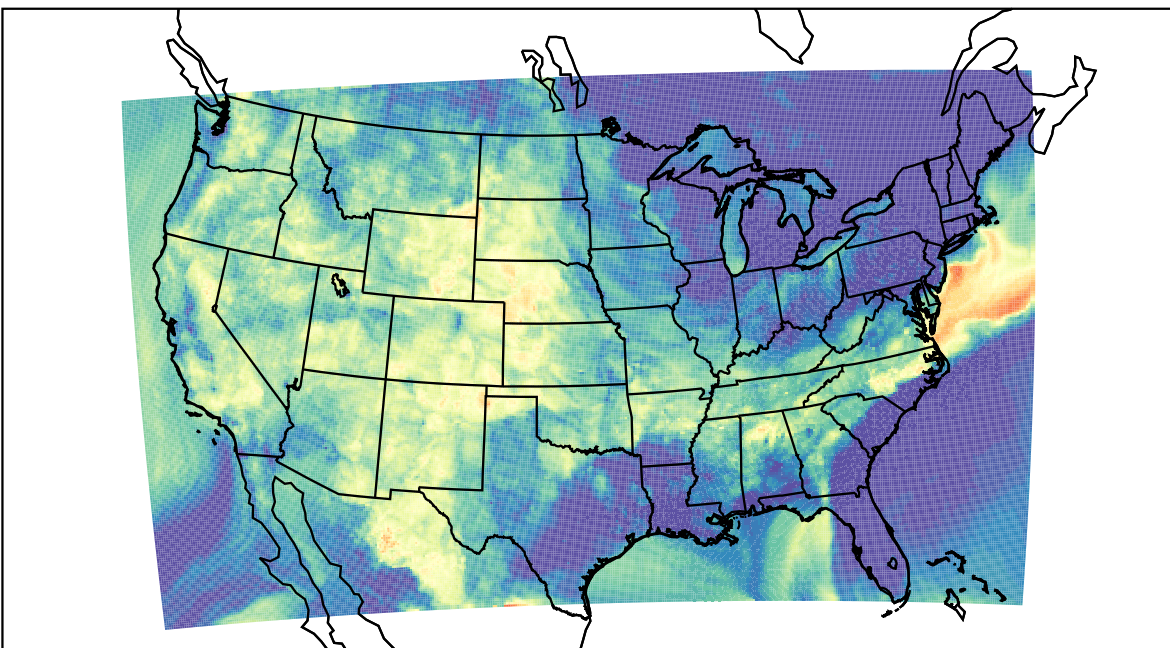
WRF (2019-08-24_05:00:00)
