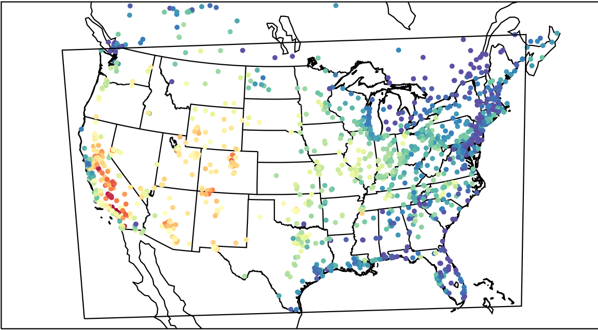
AirNOW (2019-08-23_22:00:00)
