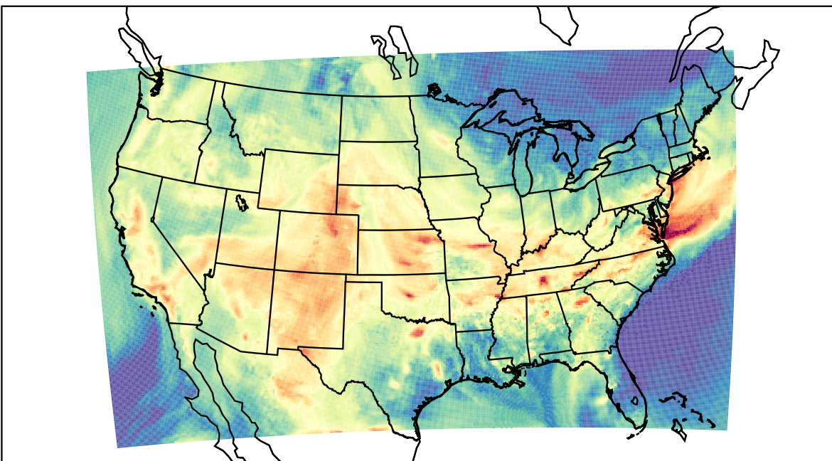
WRF (2019-08-23_21:00:00)
