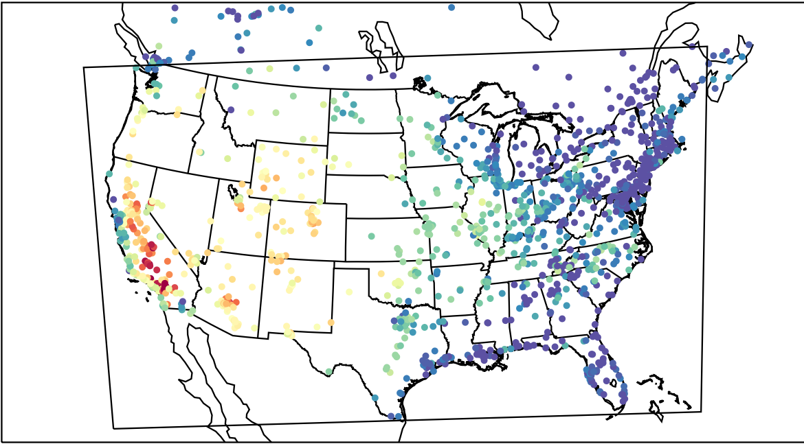
AirNOW (2019-08-24_00:00:00)
