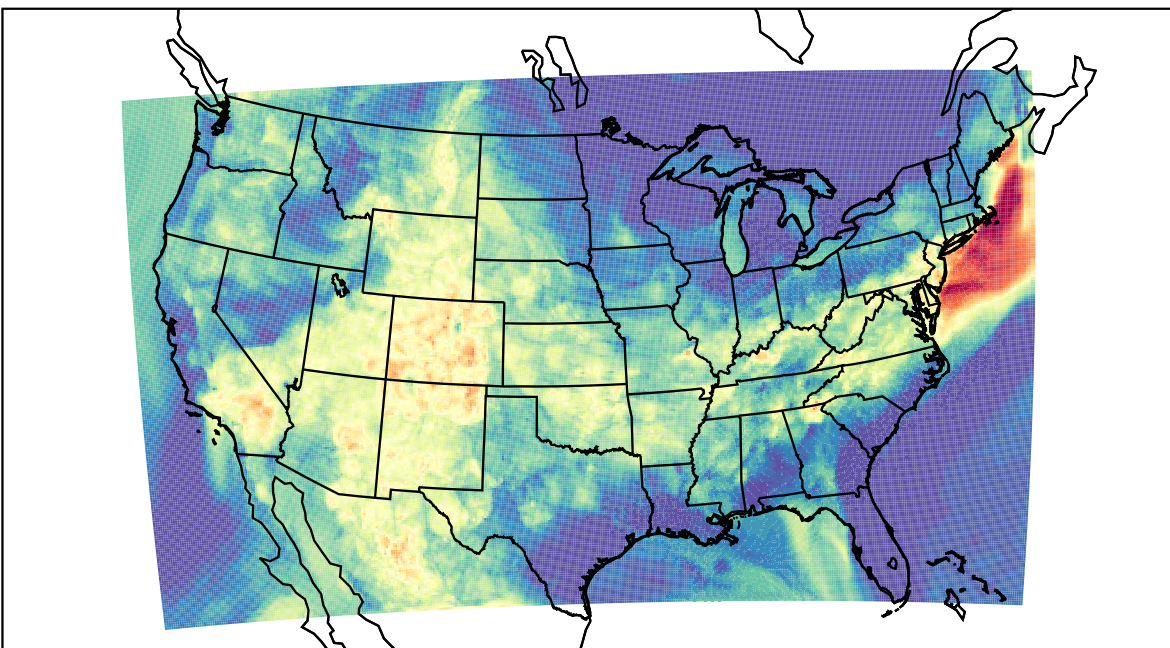
WRF (2019-08-23_04:00:00)
