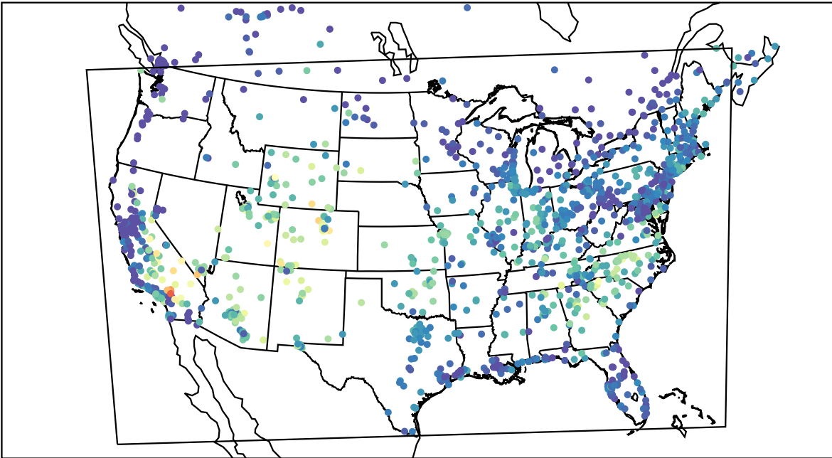
AirNOW (2019-08-23_15:00:00)
