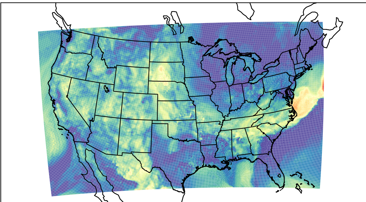
WRF (2019-08-24_14:00:00)
