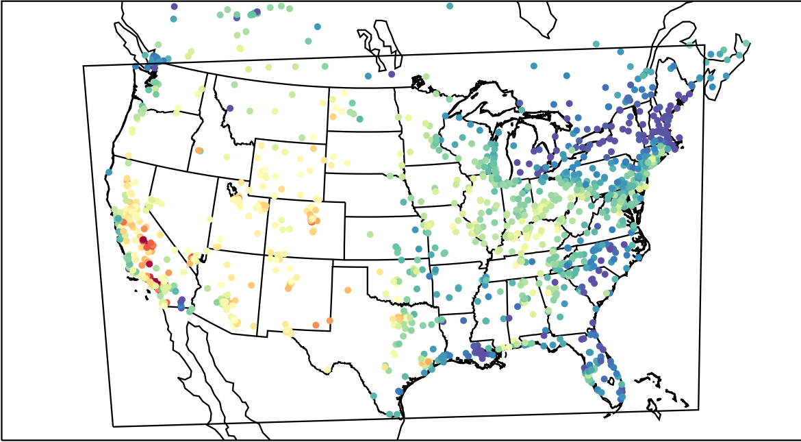
AirNOW (2019-08-24_20:00:00)
