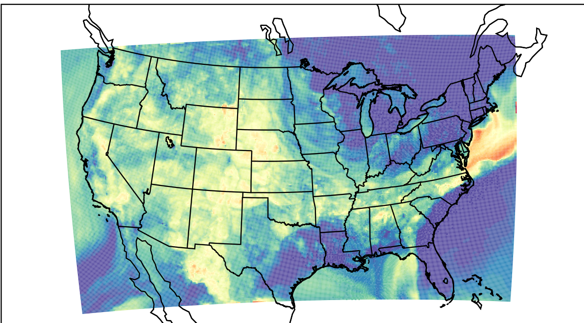
WRF (2019-08-24_04:00:00)
