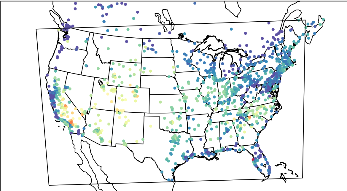
AirNOW (2019-08-23_16:00:00)
