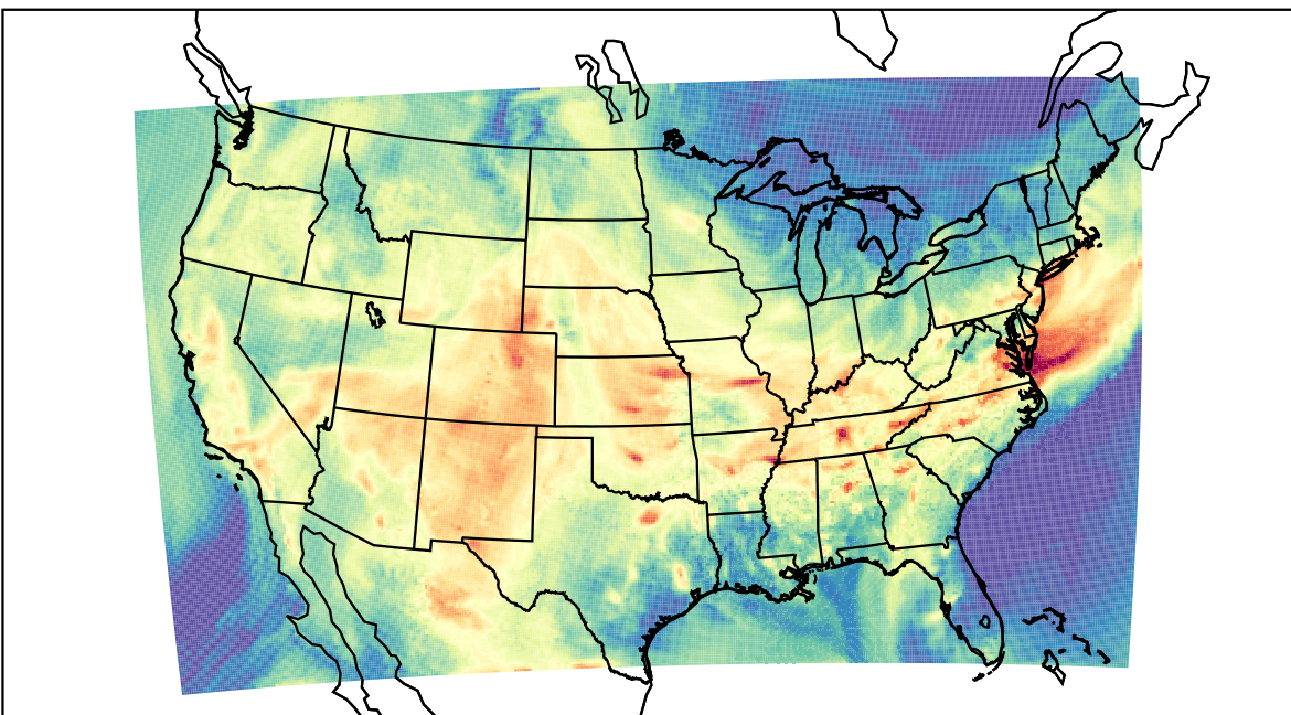
WRF (2019-08-23_20:00:00)
