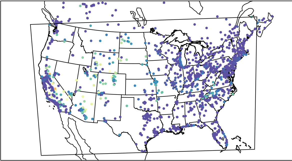
AirNOW (2019-08-24_13:00:00)
