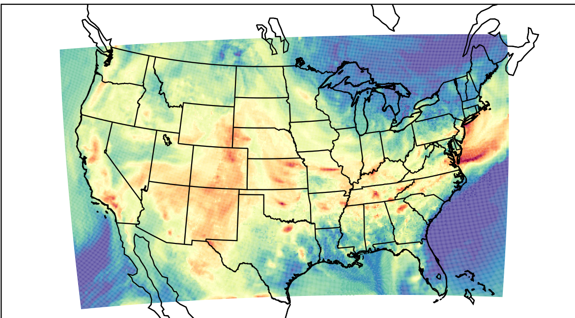
WRF (2019-08-23_22:00:00)
