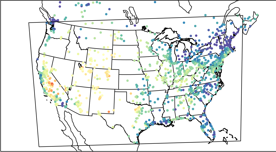
AirNOW (2019-08-24_18:00:00)
