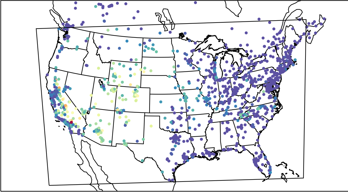
AirNOW (2019-08-24_07:00:00)
