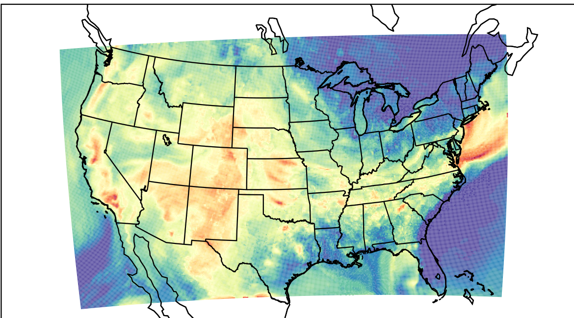
WRF (2019-08-24_00:00:00)
