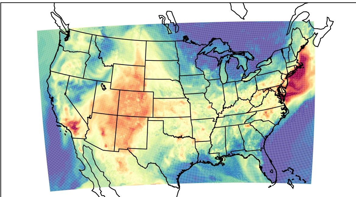
WRF (2019-08-23_00:00:00)
