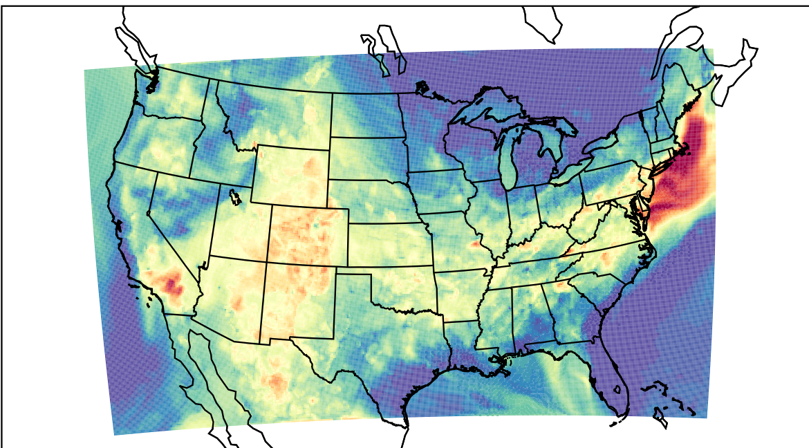
WRF (2019-08-23_02:00:00)
