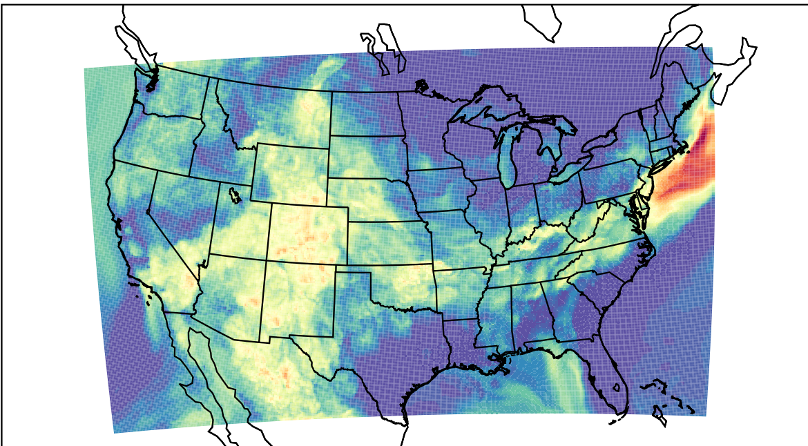
WRF (2019-08-23_07:00:00)
