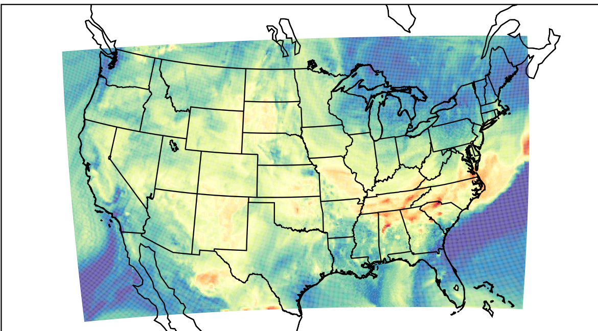
WRF (2019-08-24_17:00:00)
