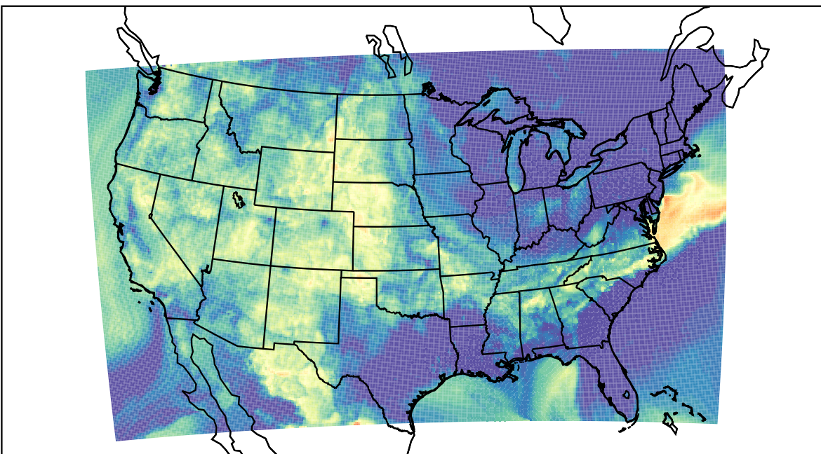
WRF (2019-08-24_08:00:00)
