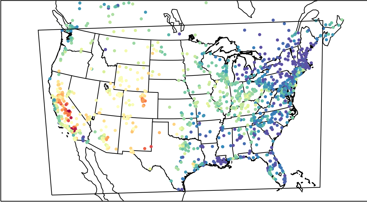
AirNOW (2019-08-24_23:00:00)
