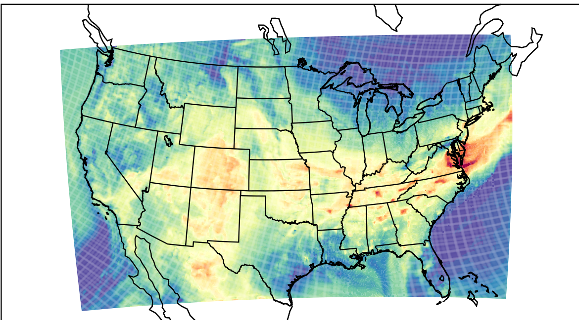
WRF (2019-08-23_17:00:00)
