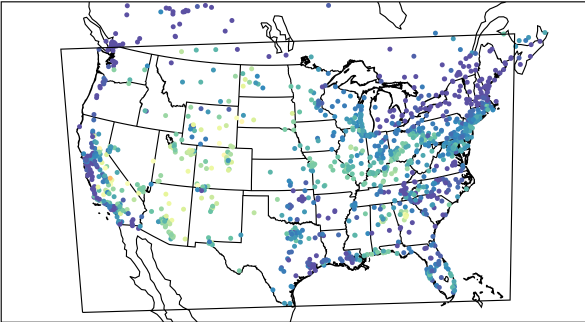
AirNOW (2019-08-24_15:00:00)
