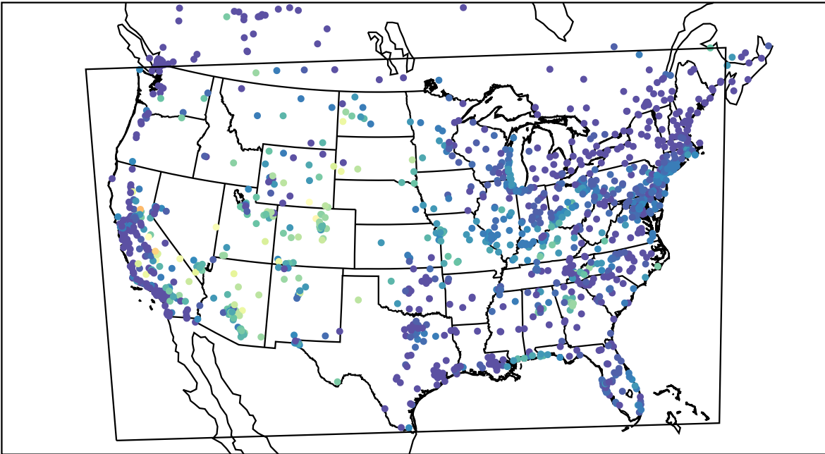
AirNOW (2019-08-24_14:00:00)
