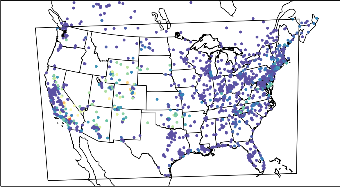
AirNOW (2019-08-23_13:00:00)
