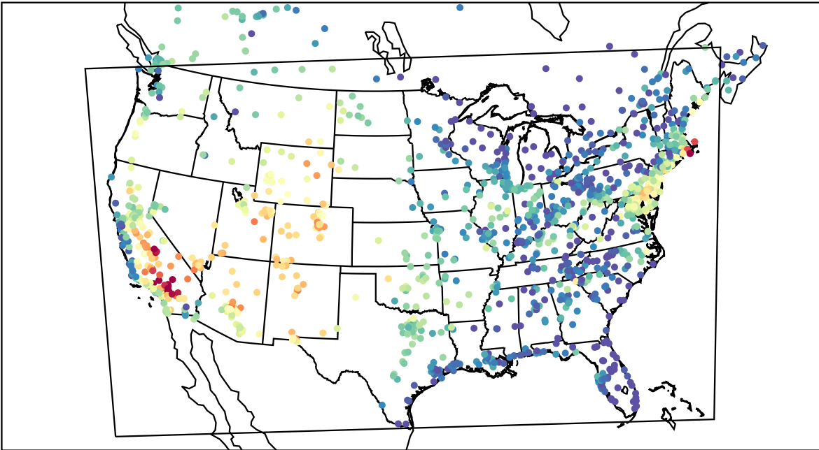
AirNOW (2019-08-23_00:00:00)
