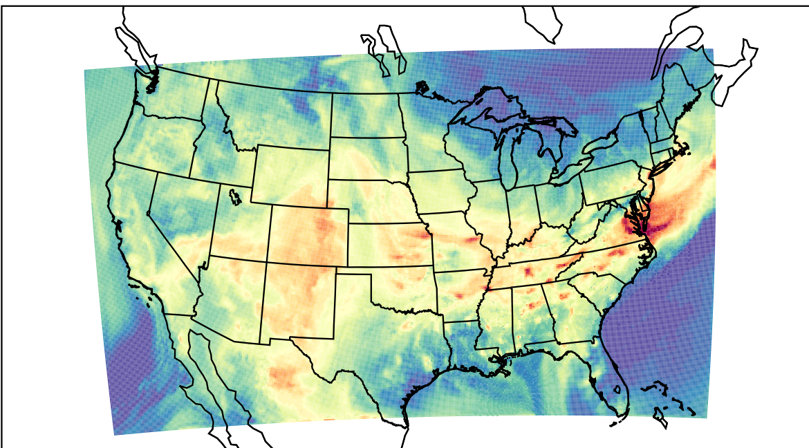
WRF (2019-08-23_18:00:00)
