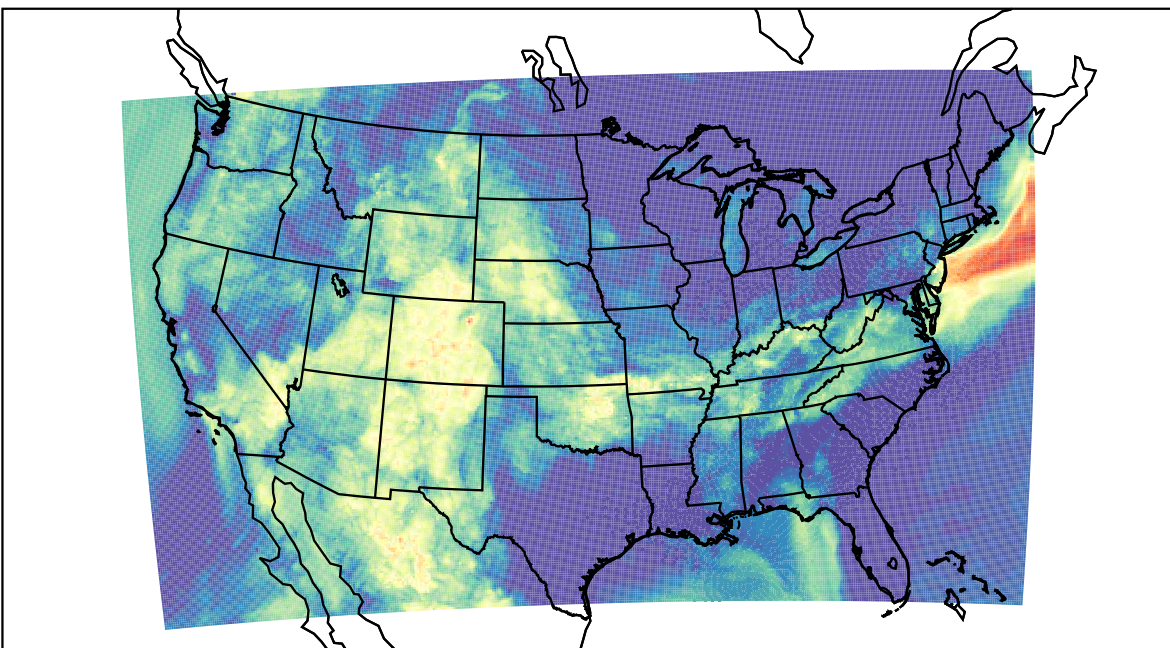
WRF (2019-08-23_10:00:00)
