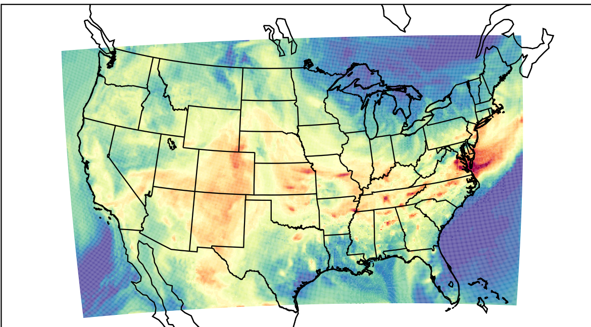
WRF (2019-08-23_19:00:00)
