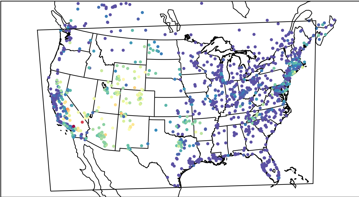
AirNOW (2019-08-23_06:00:00)
