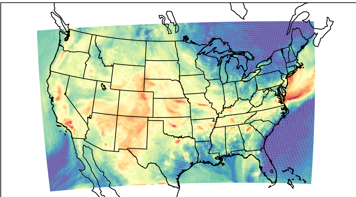
WRF (2019-08-23_23:00:00)
