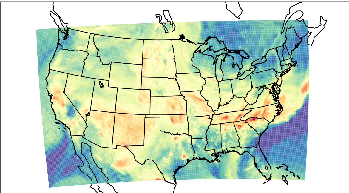
WRF (2019-08-24_21:00:00)
