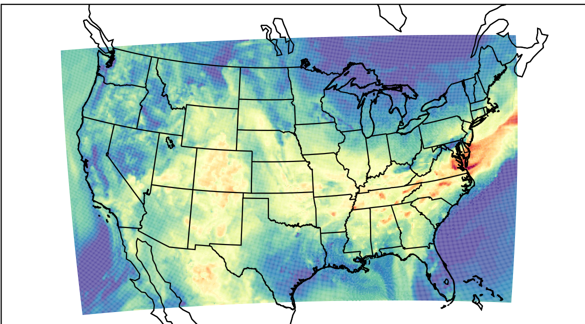
WRF (2019-08-23_16:00:00)
