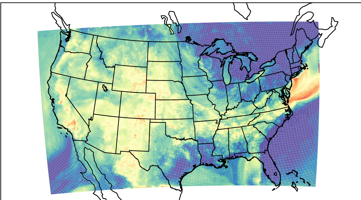
WRF (2019-08-24_02:00:00)
