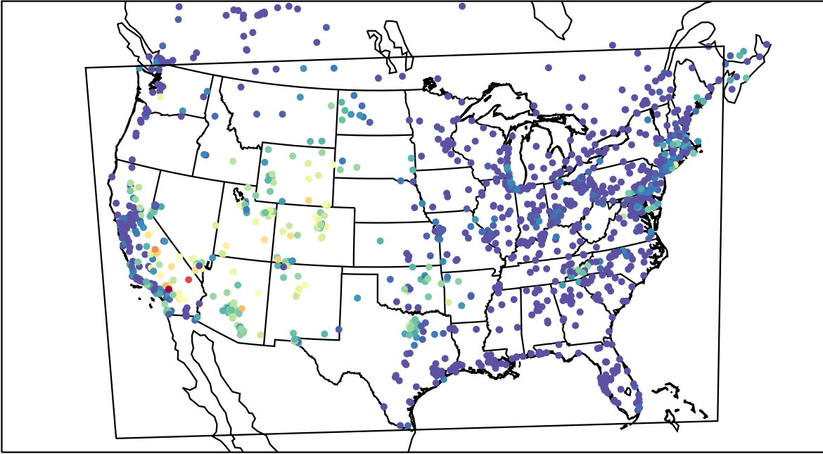
AirNOW (2019-08-23_07:00:00)
