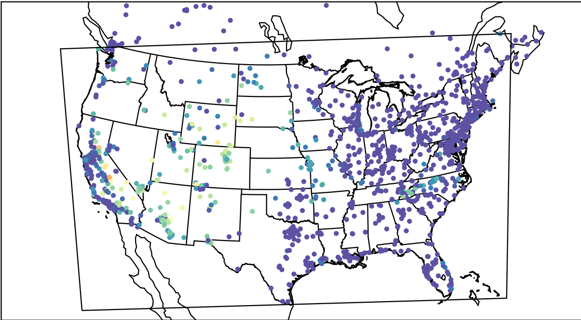
AirNOW (2019-08-24_10:00:00)
