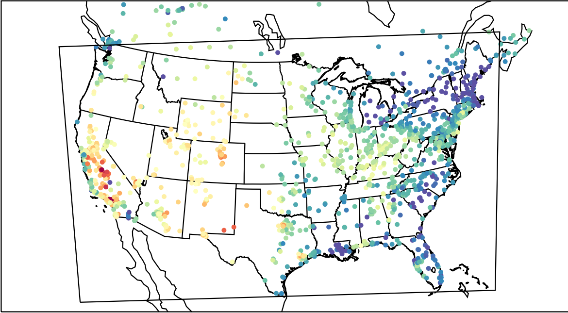
AirNOW (2019-08-24_21:00:00)
