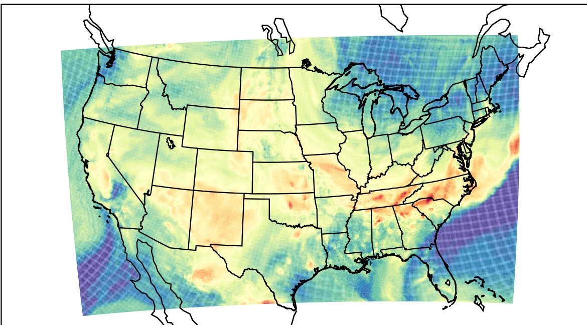
WRF (2019-08-24_19:00:00)
