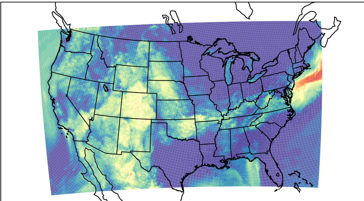
WRF (2019-08-23_12:00:00)
