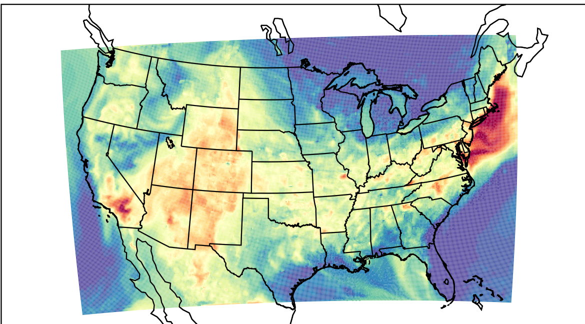
WRF (2019-08-23_01:00:00)
