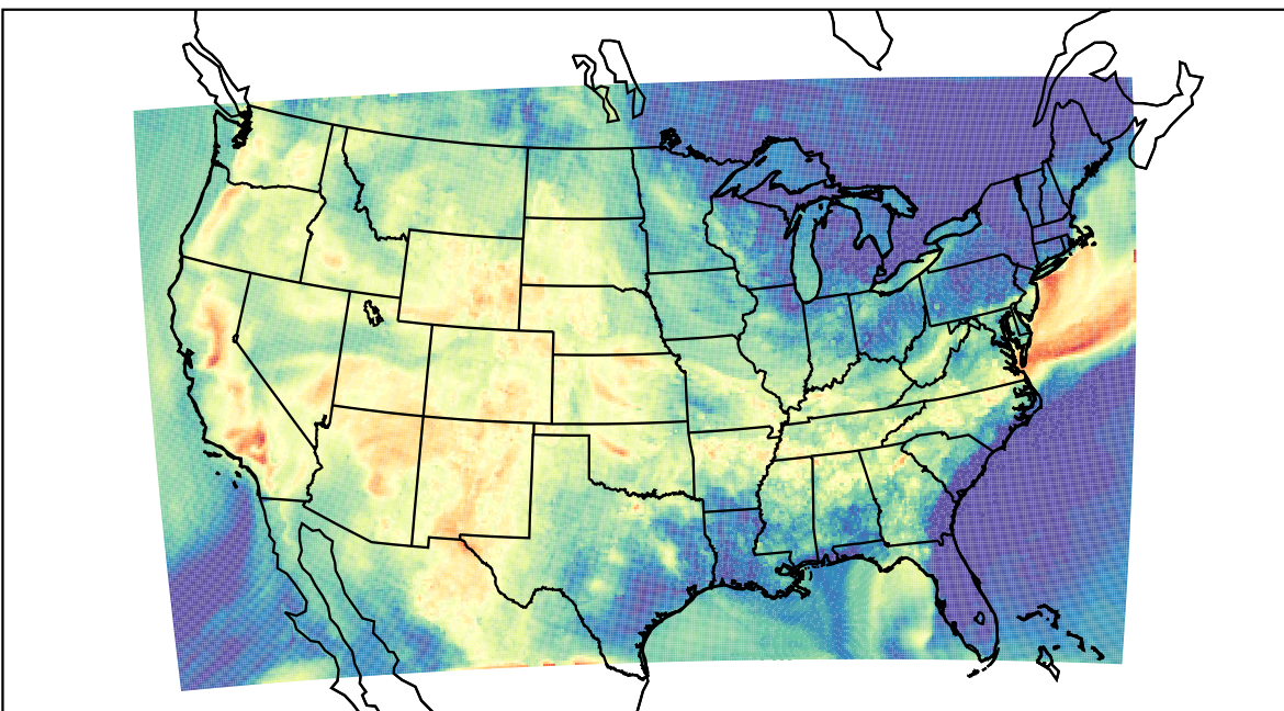
WRF (2019-08-24_01:00:00)
