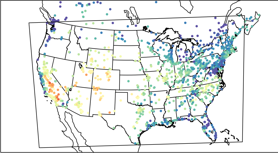
AirNOW (2019-08-23_18:00:00)
