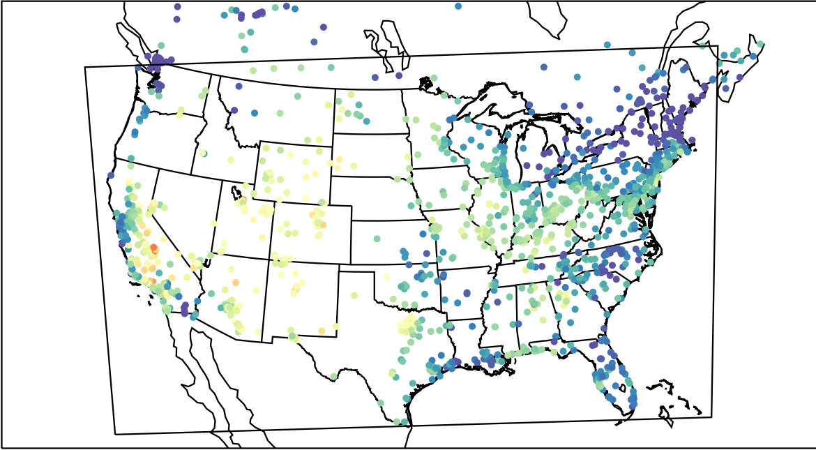
AirNOW (2019-08-24_17:00:00)
