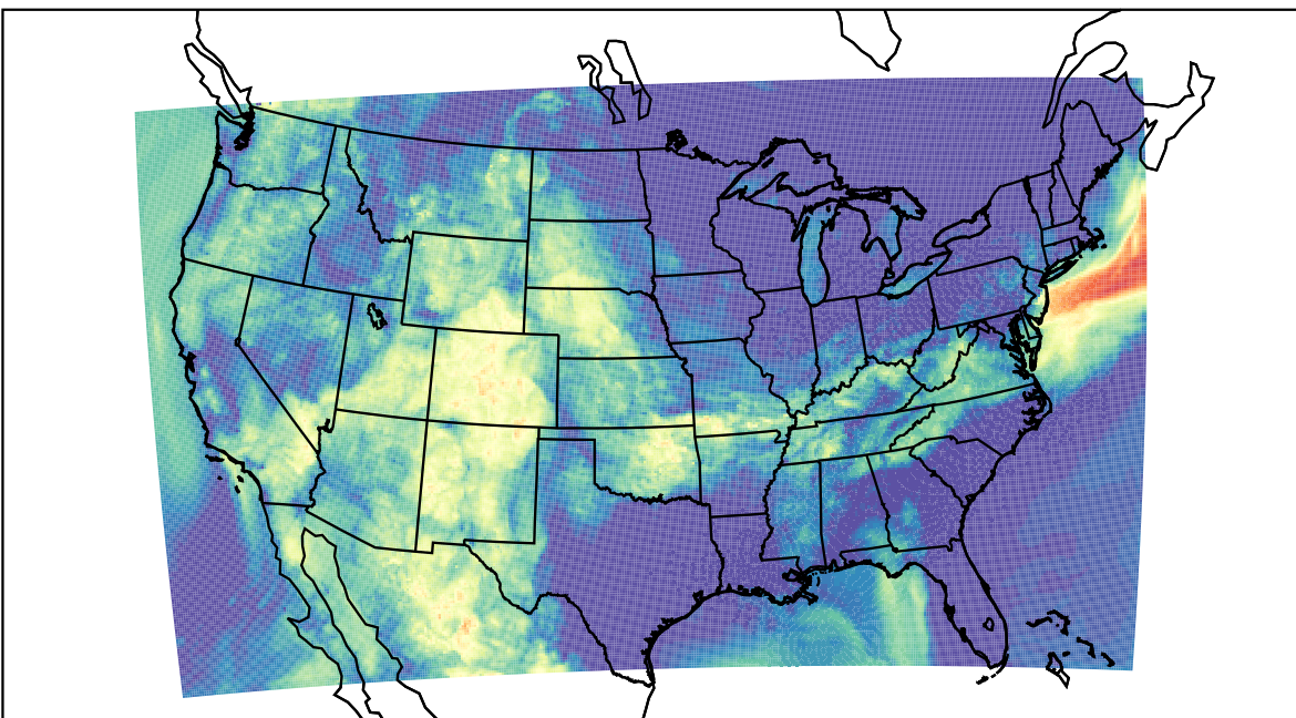
WRF (2019-08-23_11:00:00)
