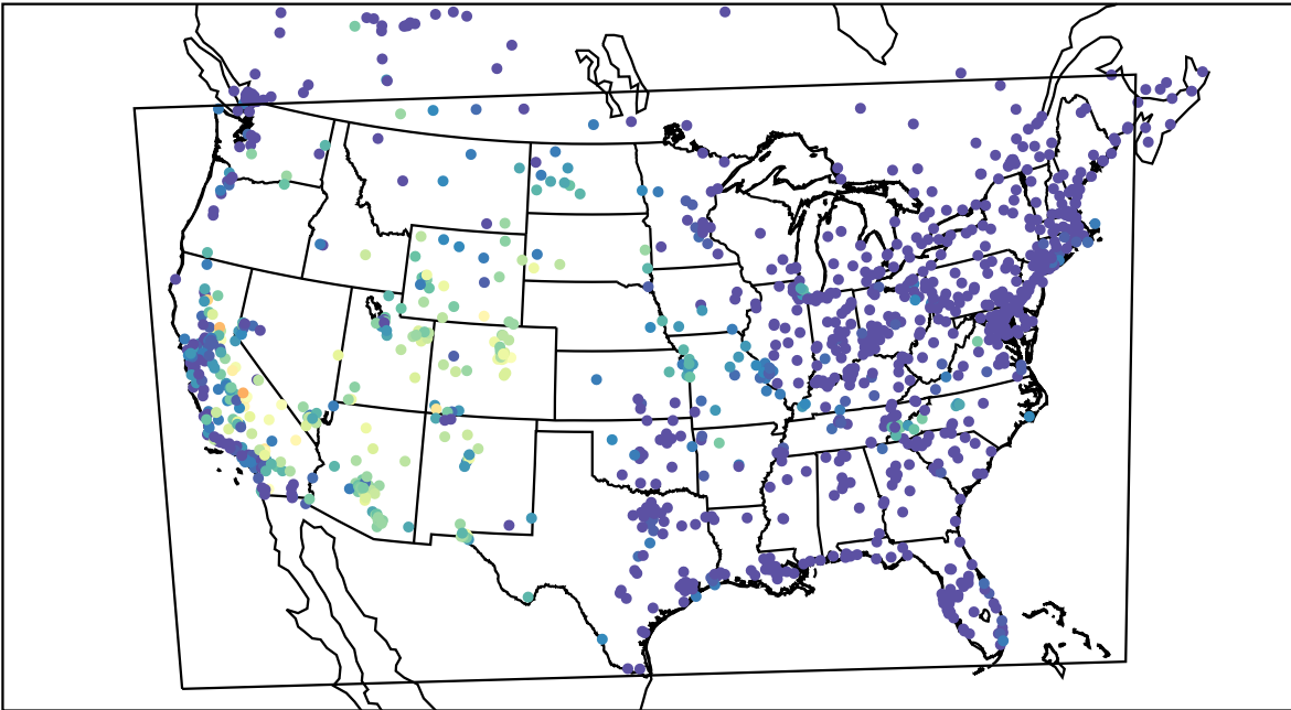
AirNOW (2019-08-24_08:00:00)
