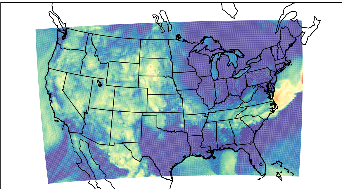
WRF (2019-08-24_13:00:00)
