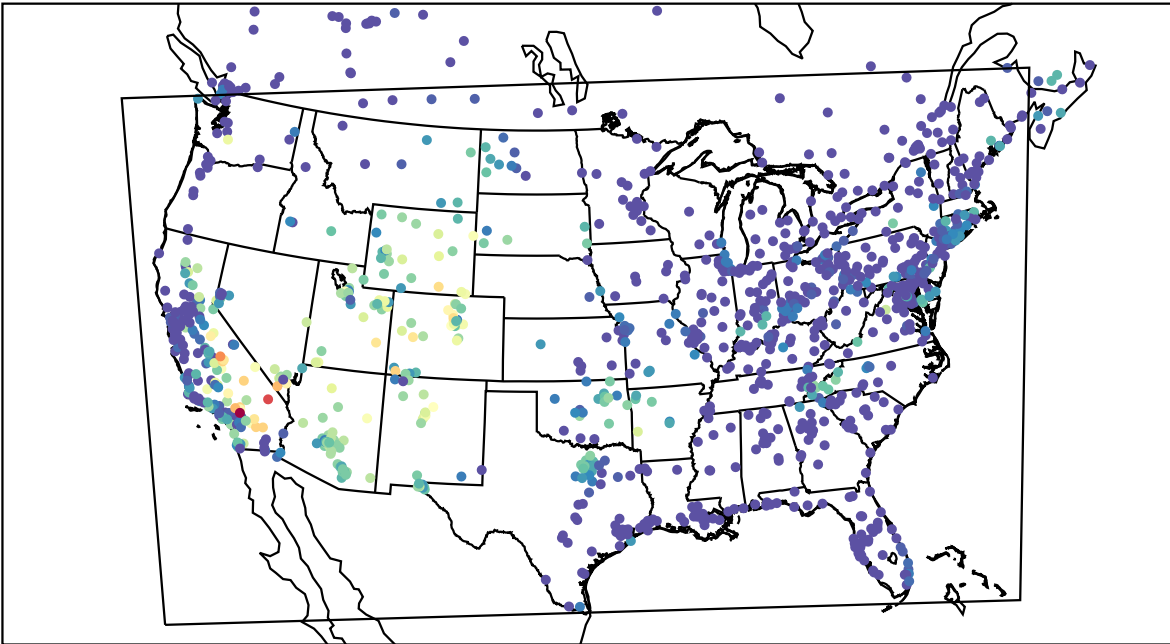
AirNOW (2019-08-23_08:00:00)
