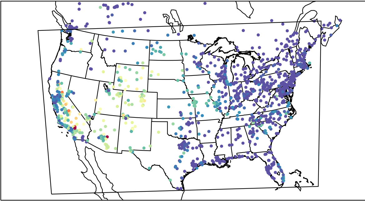
AirNOW (2019-08-24_05:00:00)
