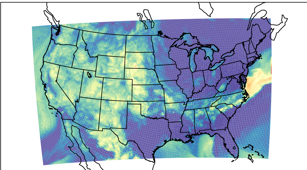
WRF (2019-08-24_11:00:00)
