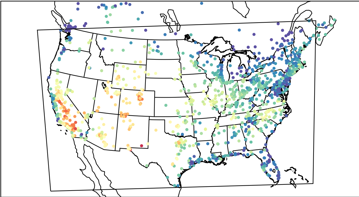
AirNOW (2019-08-23_19:00:00)
