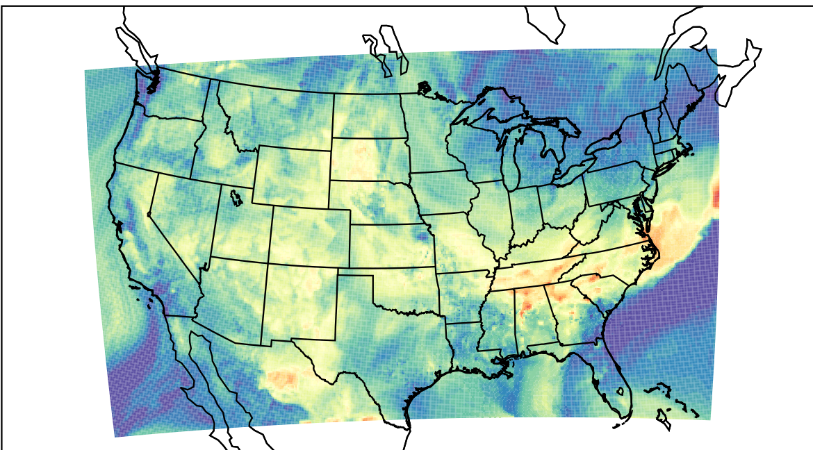
WRF (2019-08-24_16:00:00)
