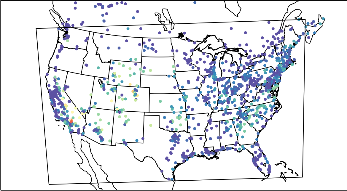
AirNOW (2019-08-23_14:00:00)
