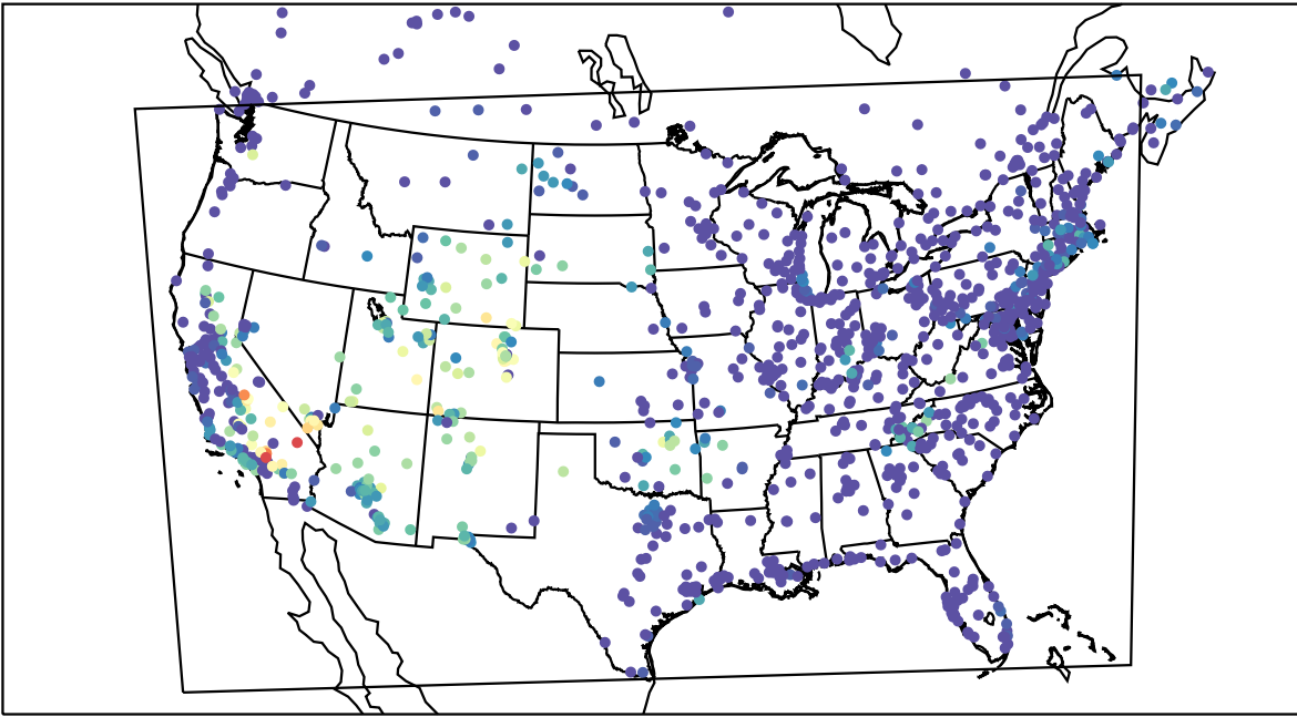
AirNOW (2019-08-23_10:00:00)
