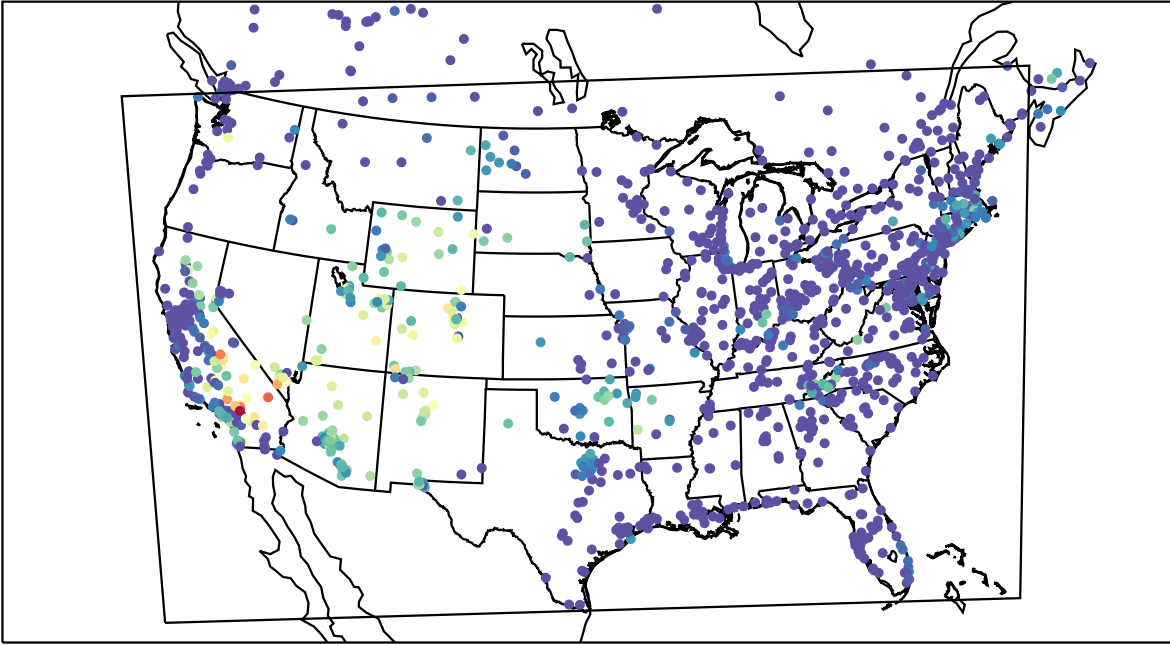
AirNOW (2019-08-23_09:00:00)
