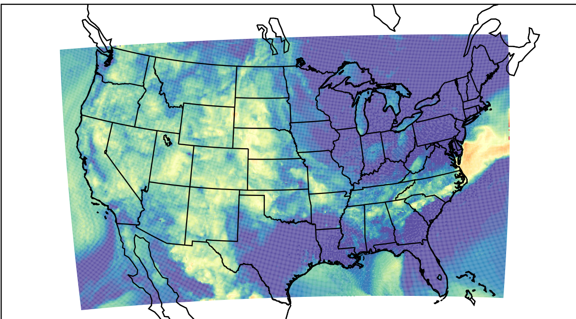
WRF (2019-08-24_10:00:00)
