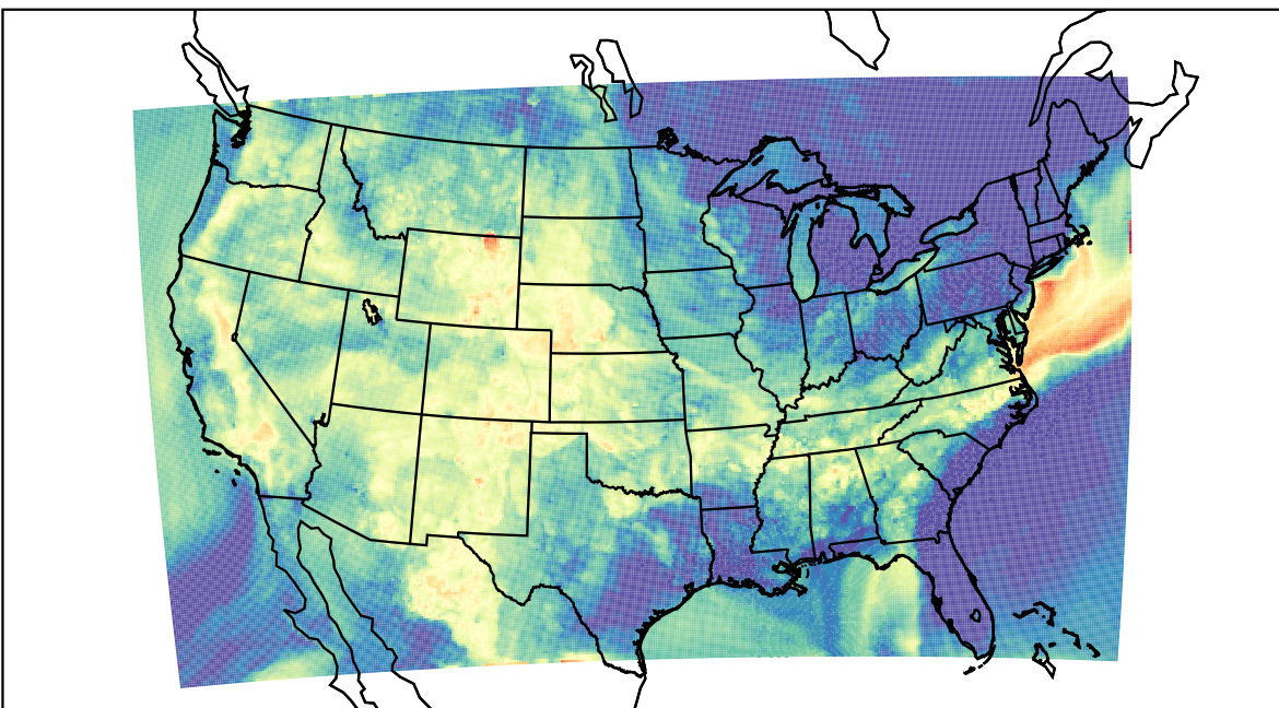
WRF (2019-08-24_03:00:00)
