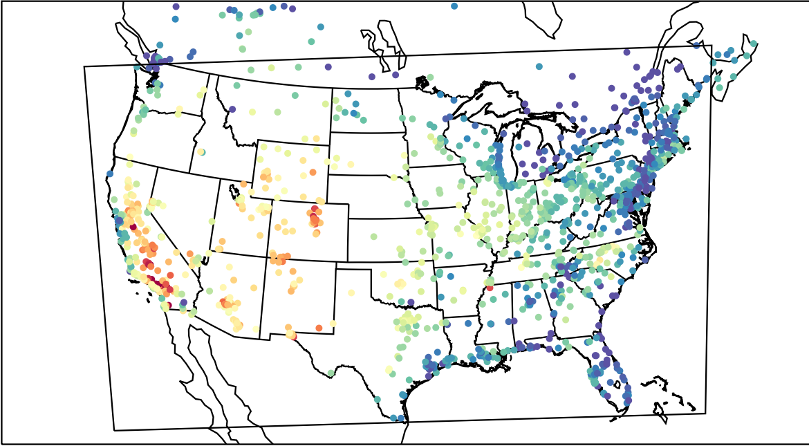
AirNOW (2019-08-23_21:00:00)
