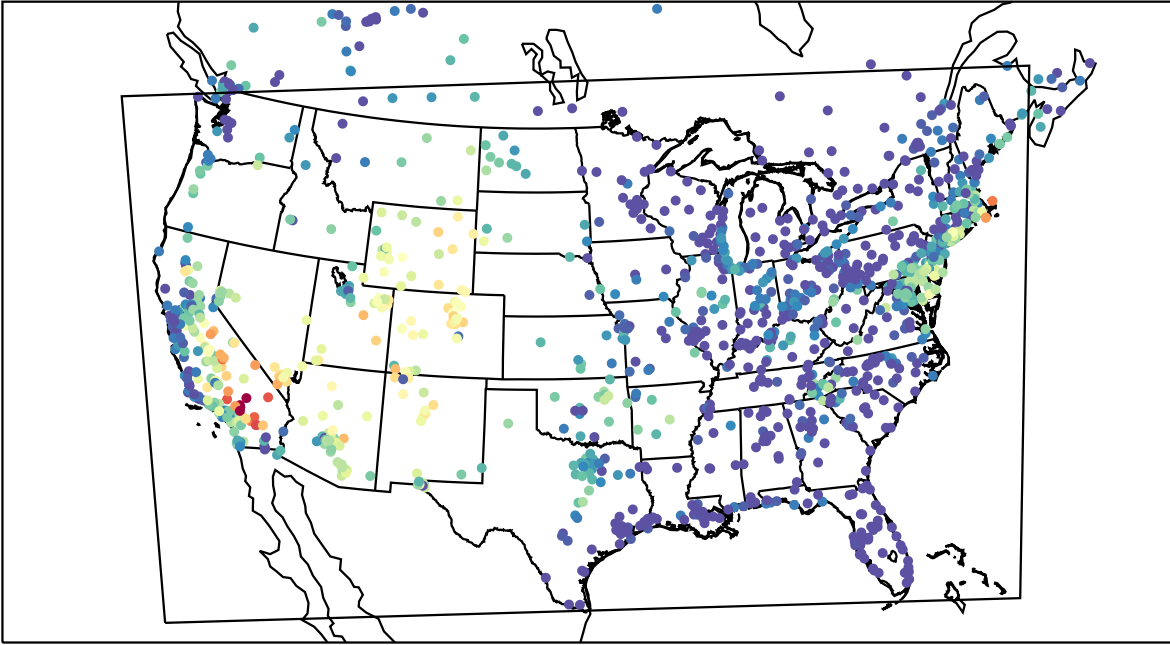
AirNOW (2019-08-23_03:00:00)
