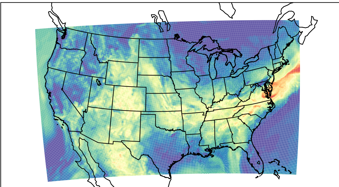
WRF (2019-08-23_15:00:00)
