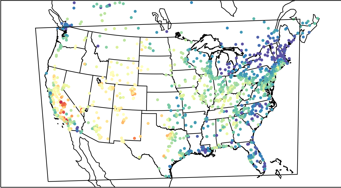
AirNOW (2019-08-24_19:00:00)
