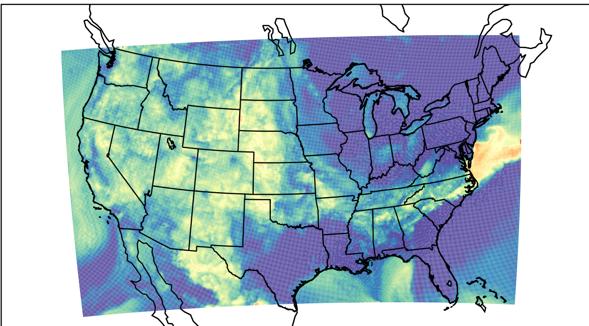
WRF (2019-08-24_09:00:00)
