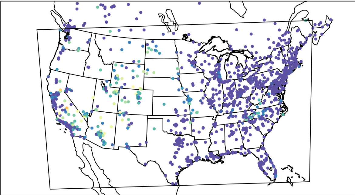
AirNOW (2019-08-24_12:00:00)
