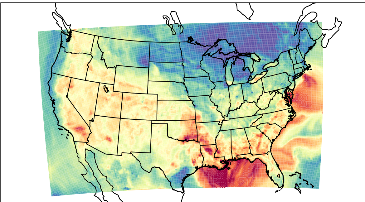
WRF (2019-09-08_01:00:00)
