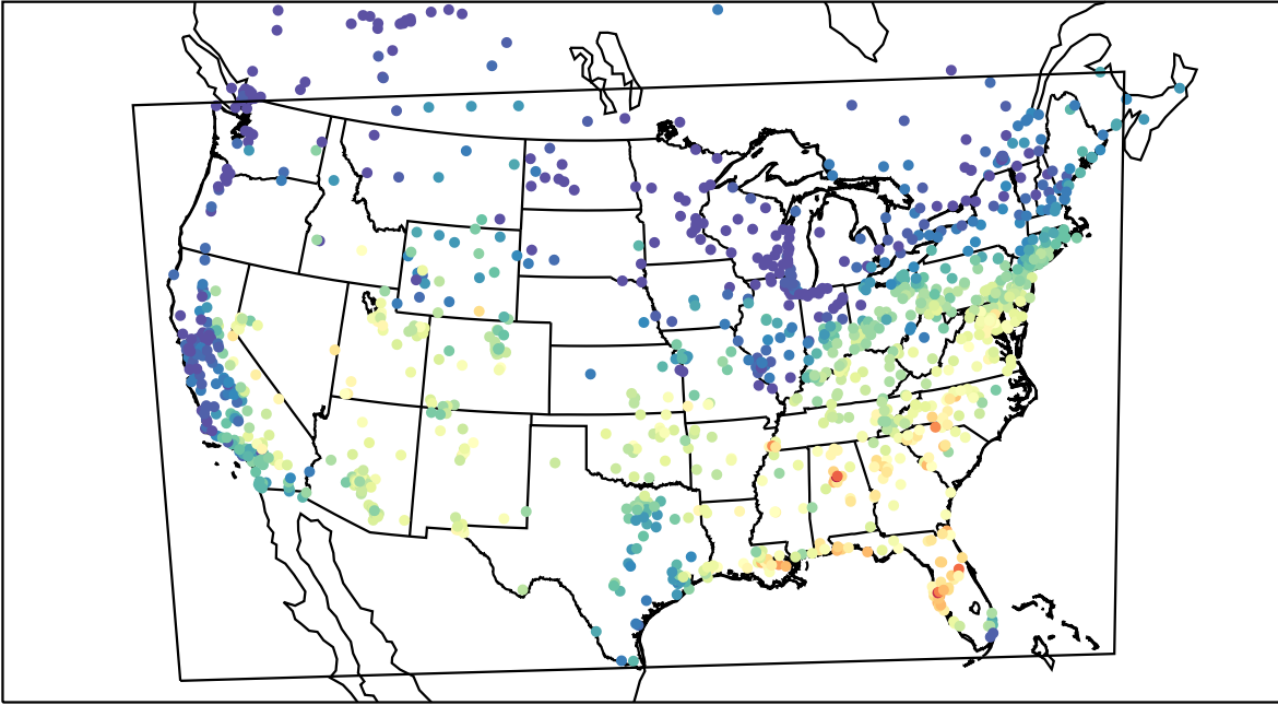
AirNOW (2019-09-08_16:00:00)
