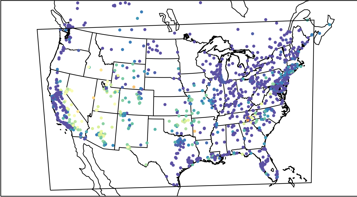
AirNOW (2019-09-08_10:00:00)
