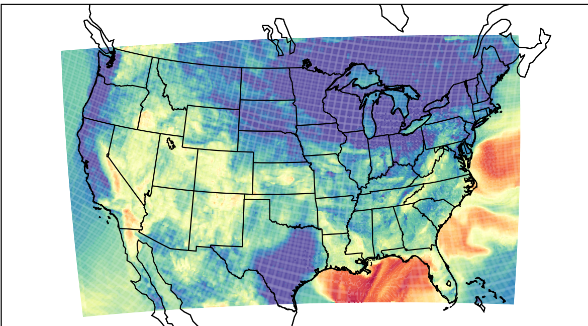
WRF (2019-09-08_11:00:00)
