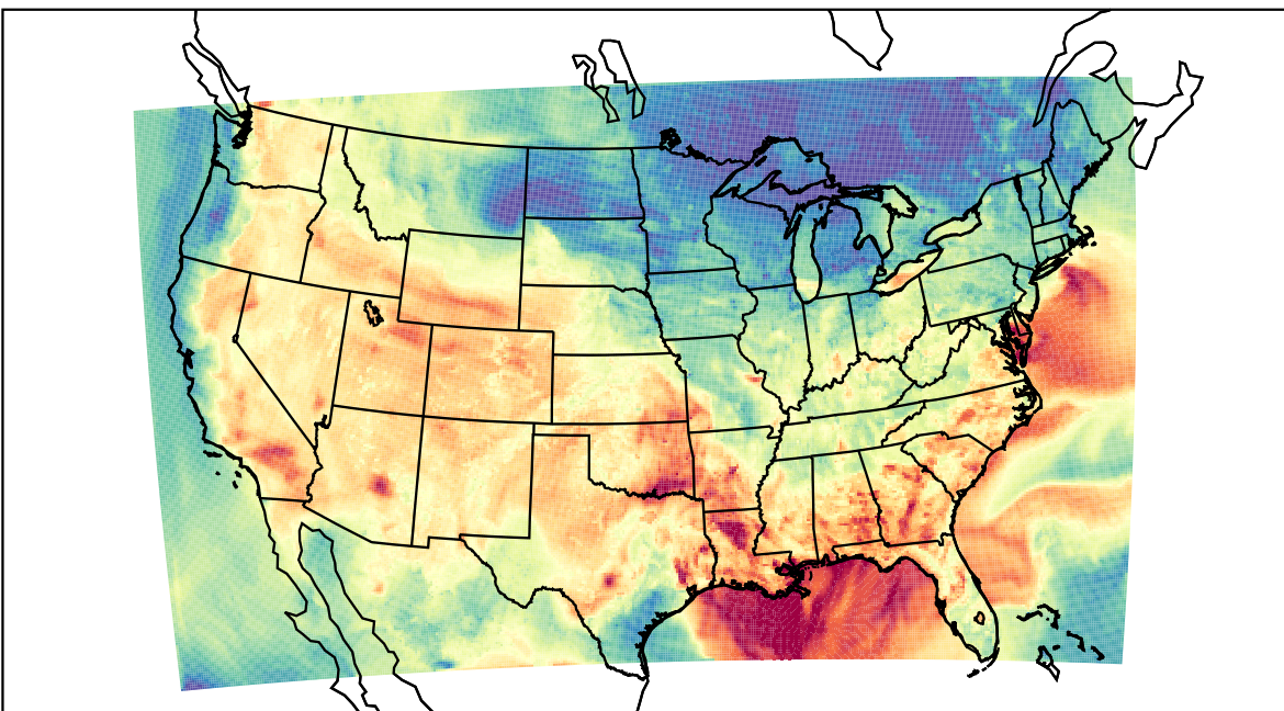
WRF (2019-09-08_00:00:00)
