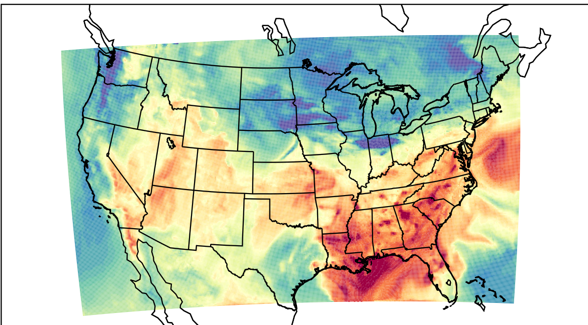
WRF (2019-09-08_18:00:00)
