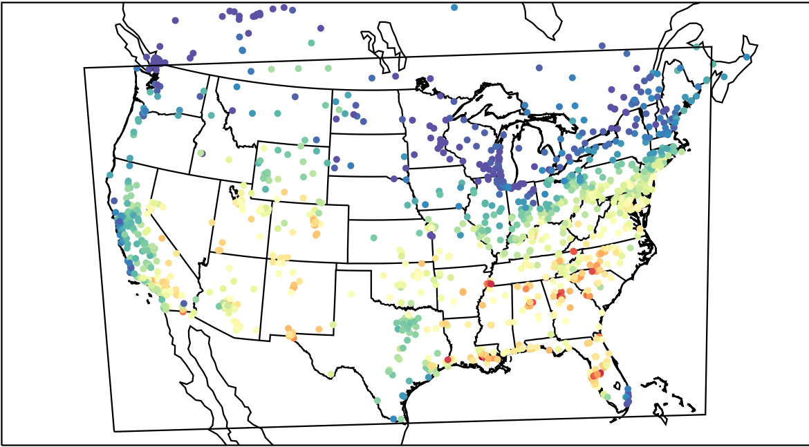
AirNOW (2019-09-08_19:00:00)
