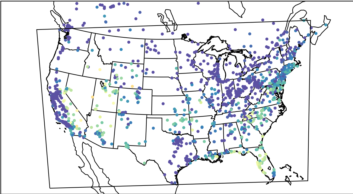
AirNOW (2019-09-08_13:00:00)
