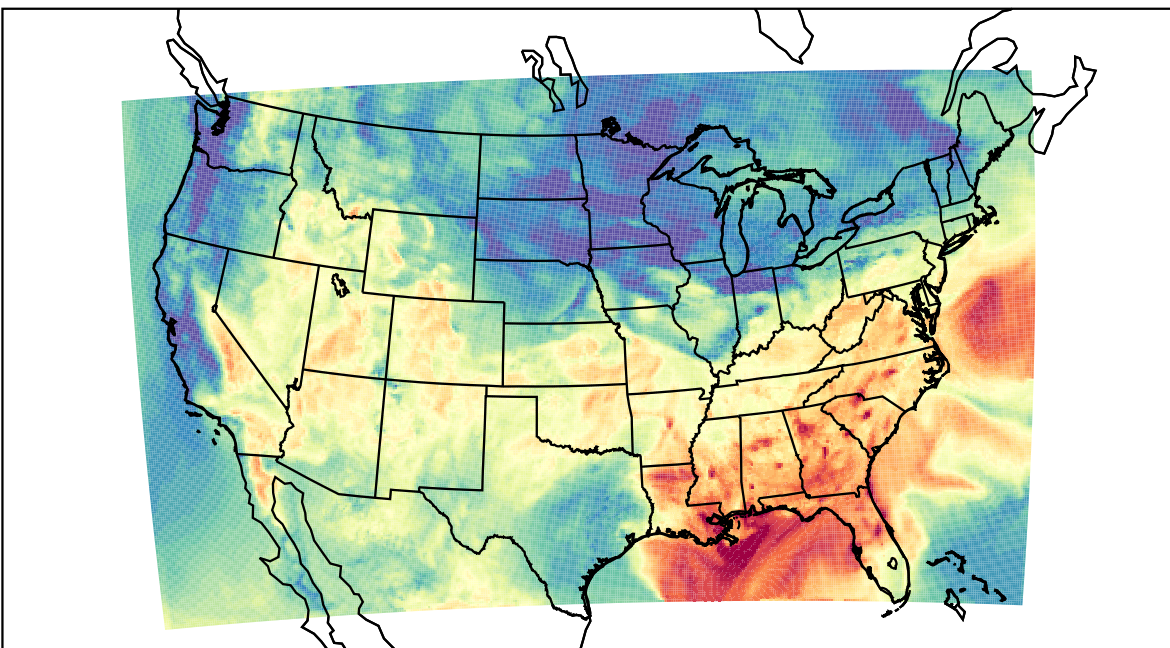
WRF (2019-09-08_16:00:00)
