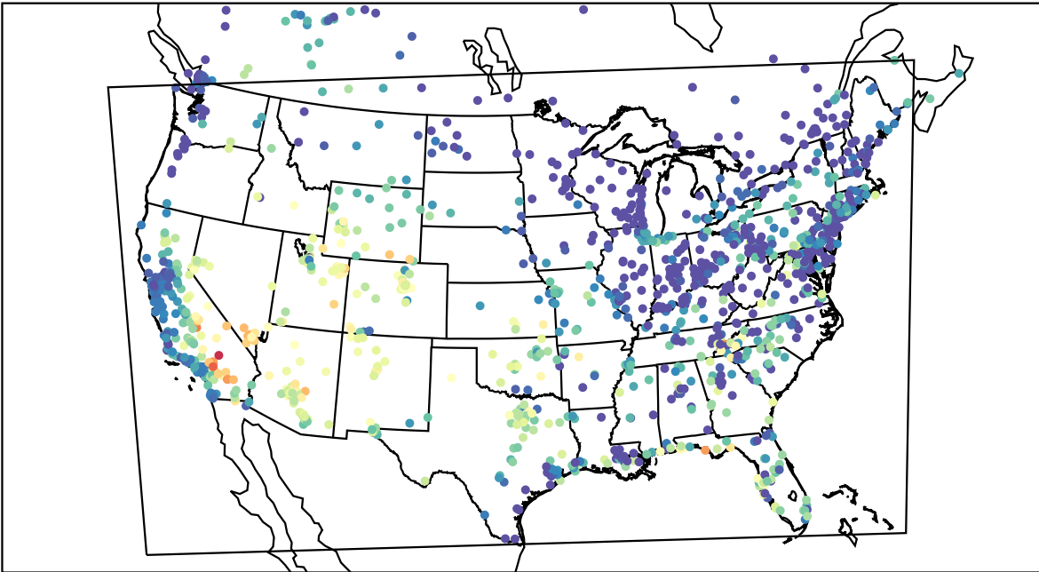
AirNOW (2019-09-08_03:00:00)
