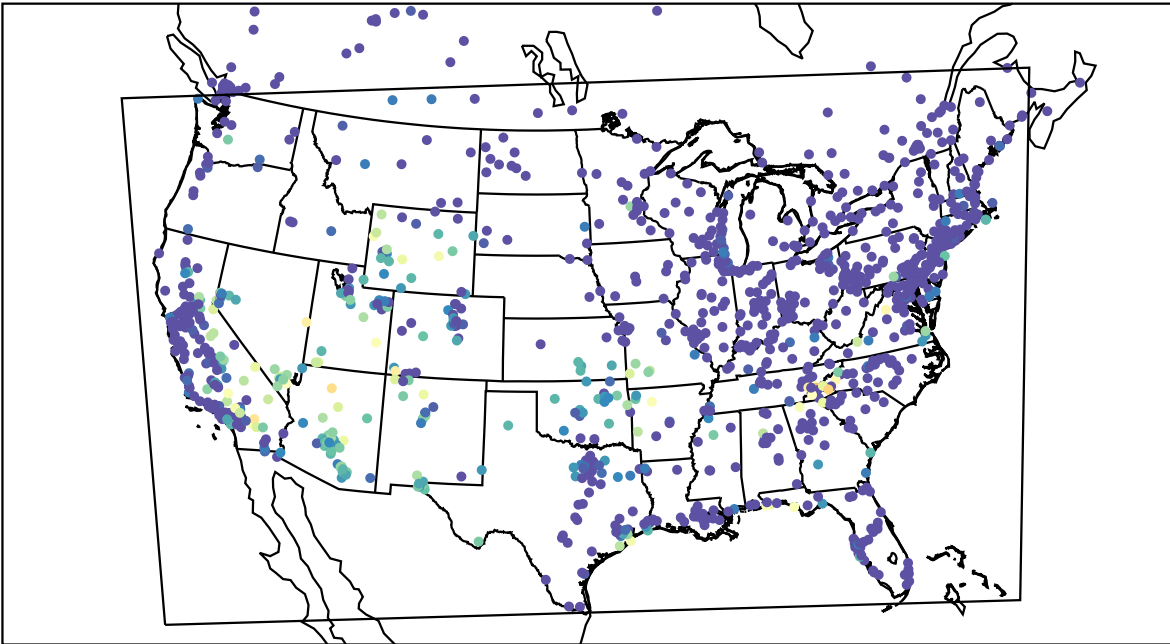
AirNOW (2019-09-09_10:00:00)
