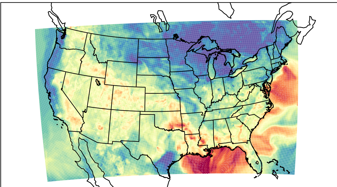
WRF (2019-09-08_03:00:00)
