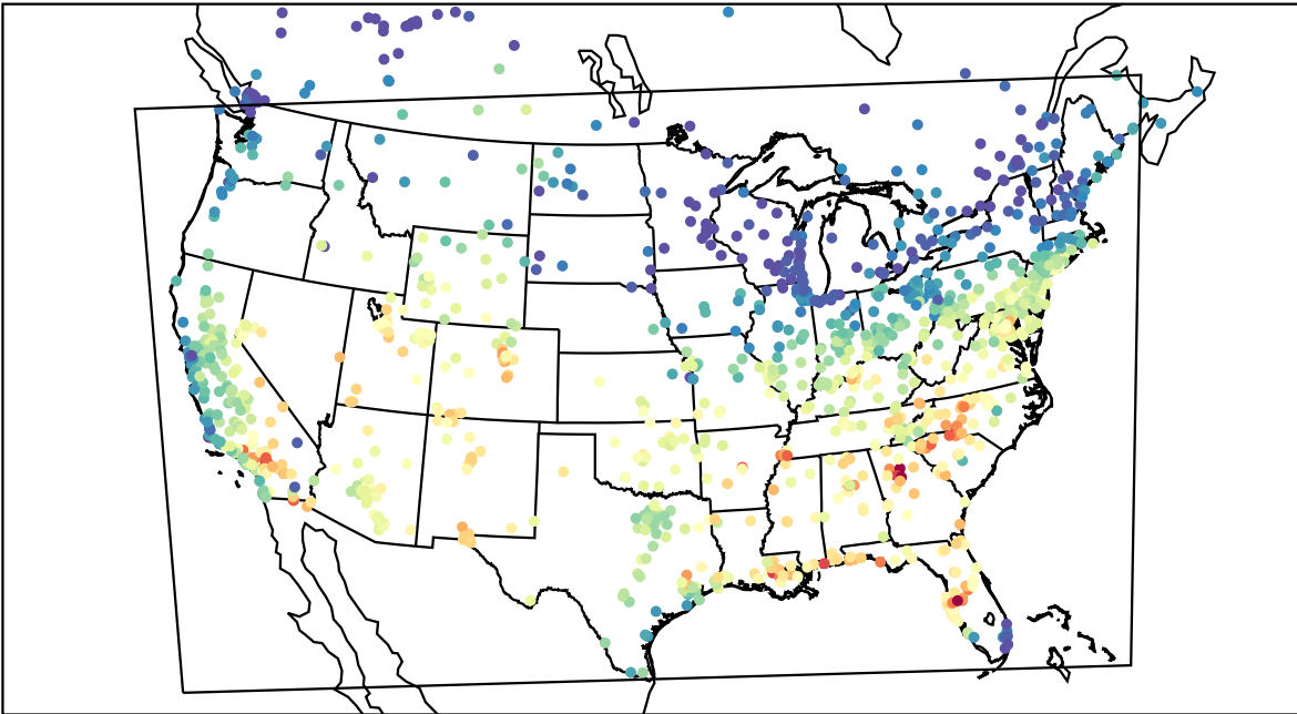
AirNOW (2019-09-08_21:00:00)
