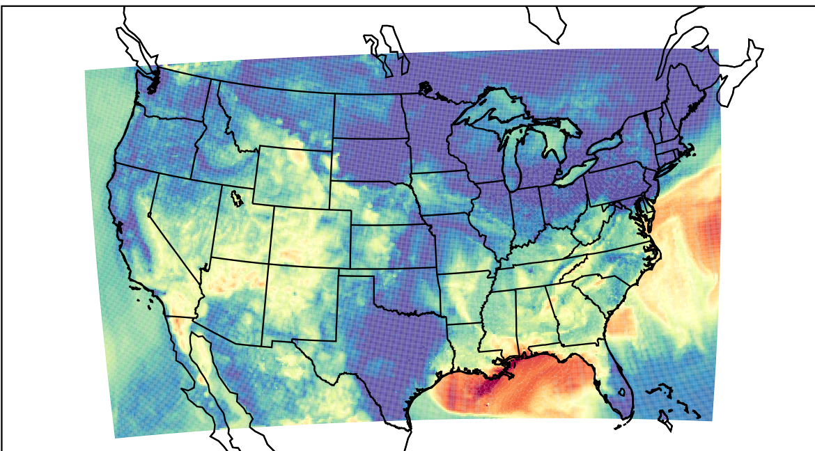
WRF (2019-09-09_11:00:00)
