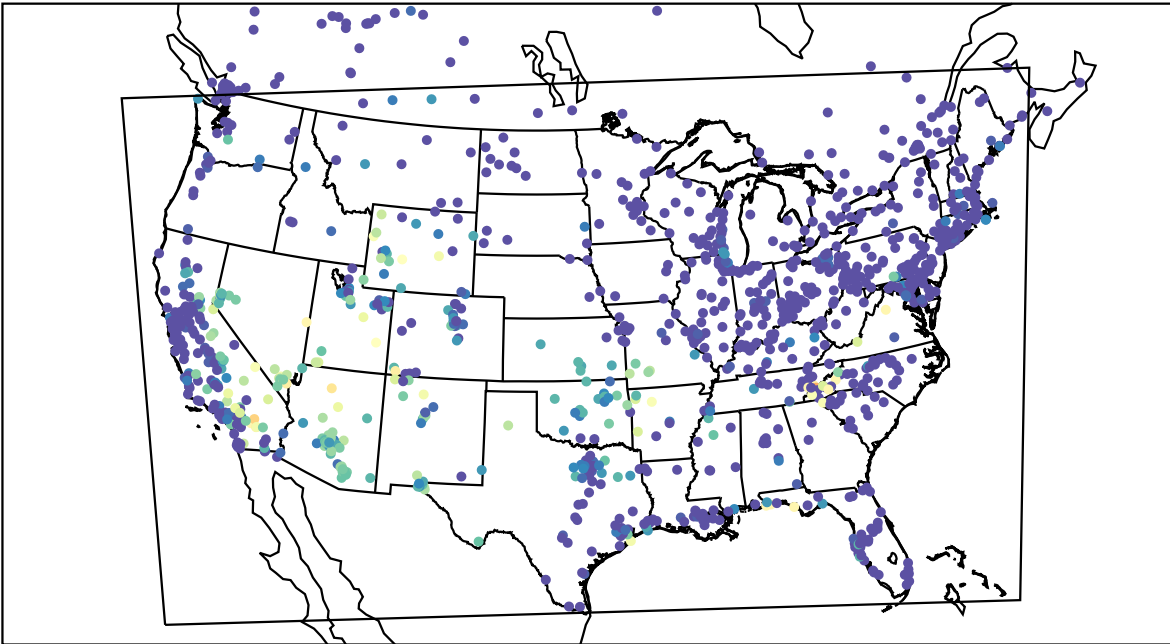
AirNOW (2019-09-09_09:00:00)
