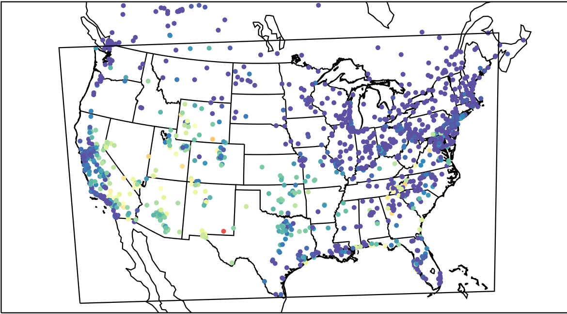
AirNOW (2019-09-09_05:00:00)
