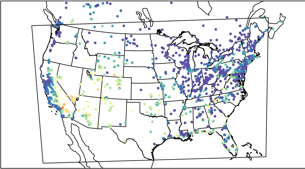
AirNOW (2019-09-08_04:00:00)
