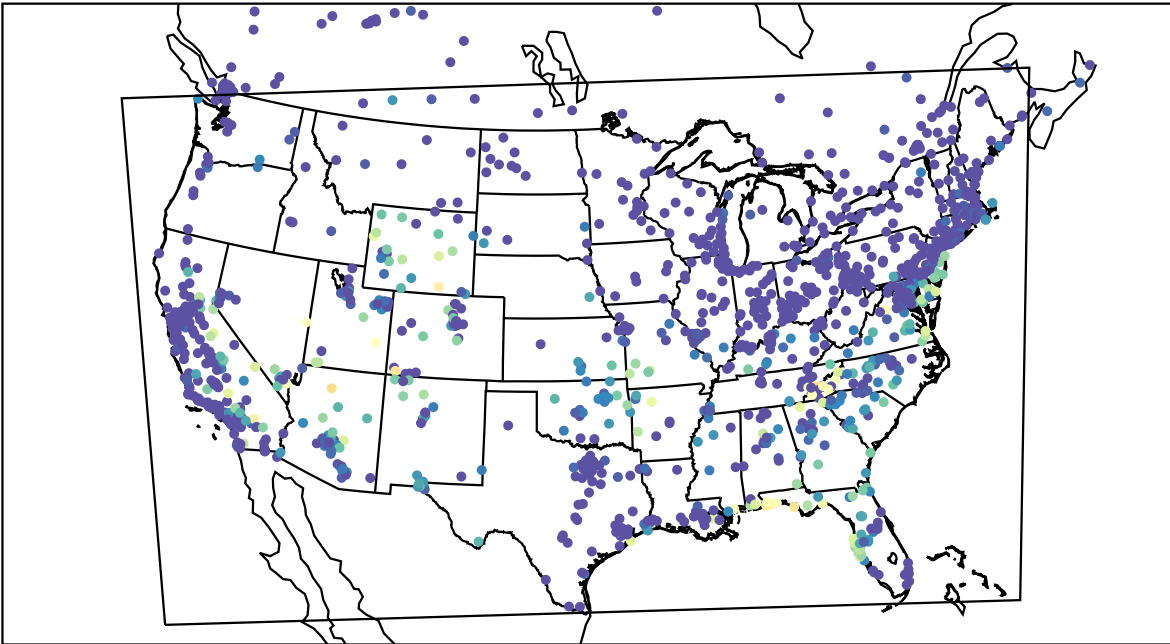
AirNOW (2019-09-09_13:00:00)
