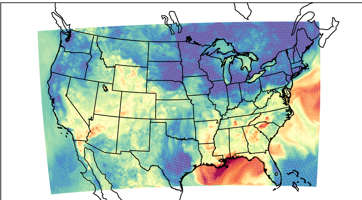
WRF (2019-09-09_05:00:00)
