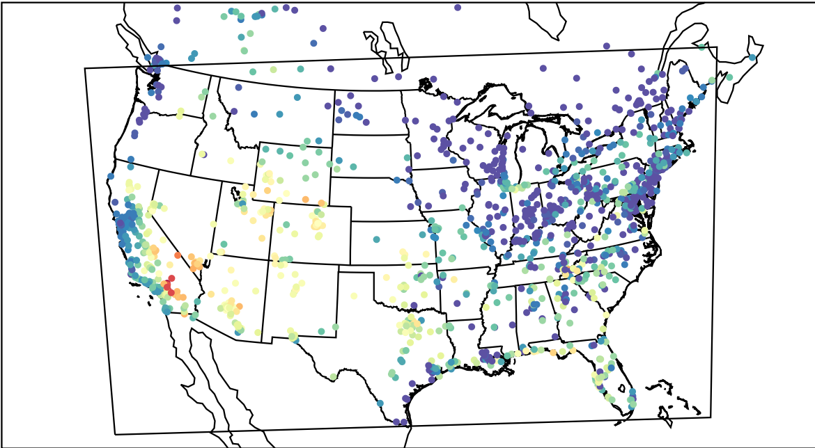
AirNOW (2019-09-08_02:00:00)
