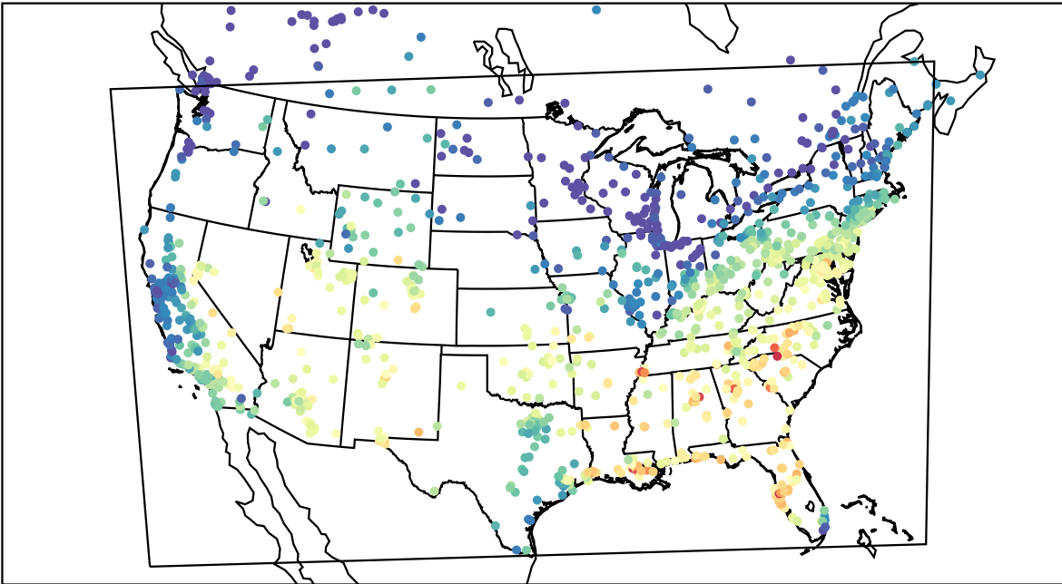
AirNOW (2019-09-08_17:00:00)
