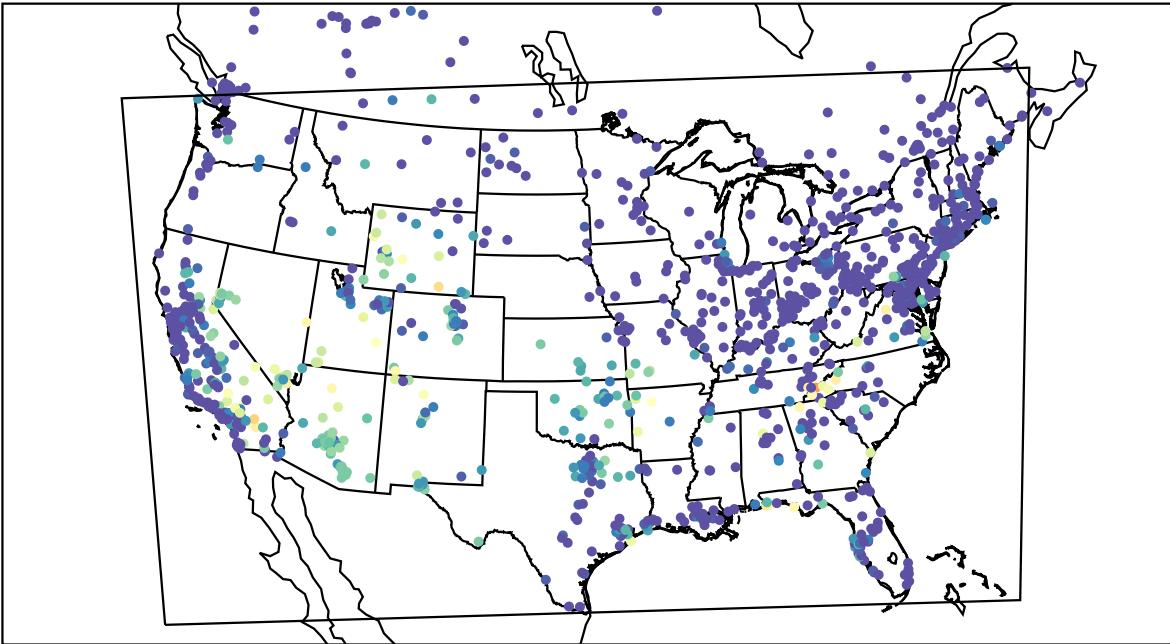
AirNOW (2019-09-09_08:00:00)
