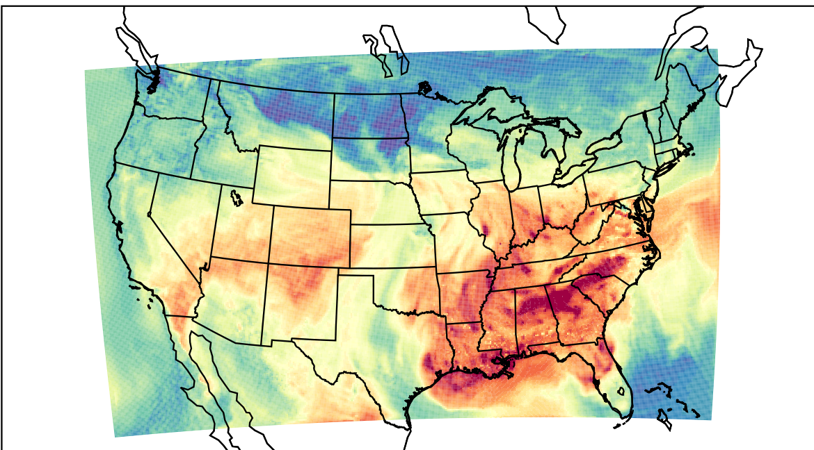
WRF (2019-09-09_19:00:00)
