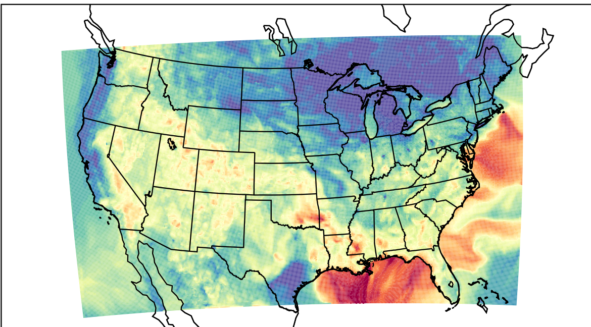
WRF (2019-09-08_04:00:00)
