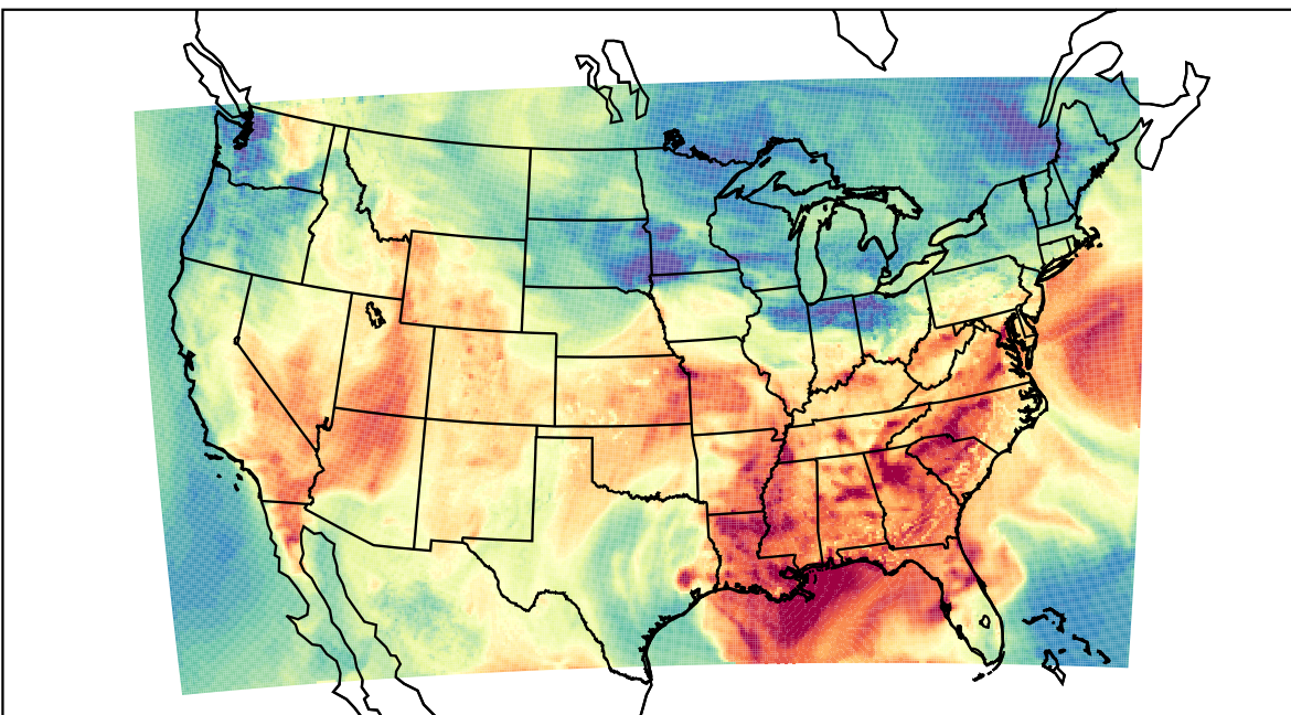
WRF (2019-09-08_21:00:00)
