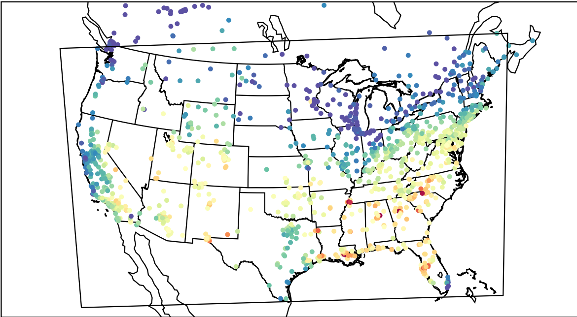
AirNOW (2019-09-08_18:00:00)
