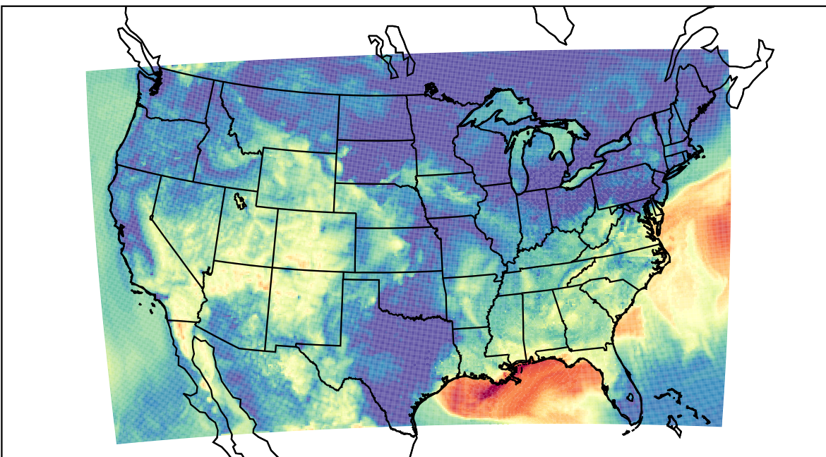
WRF (2019-09-09_13:00:00)
