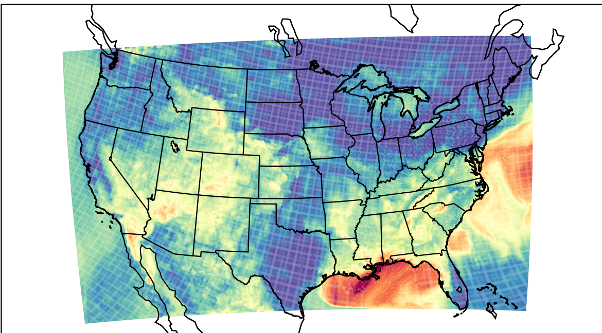
WRF (2019-09-09_09:00:00)
