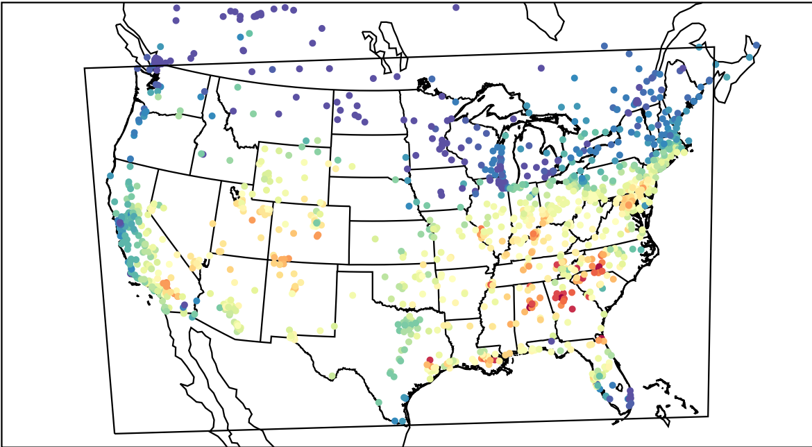
AirNOW (2019-09-09_18:00:00)
