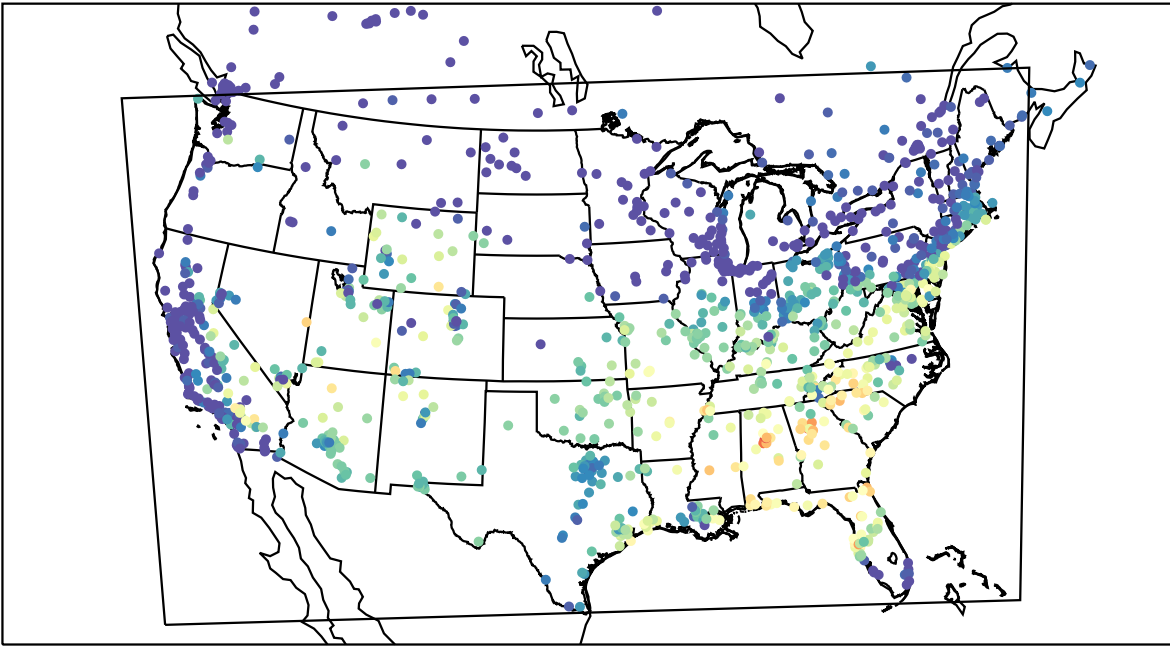
AirNOW (2019-09-09_15:00:00)
