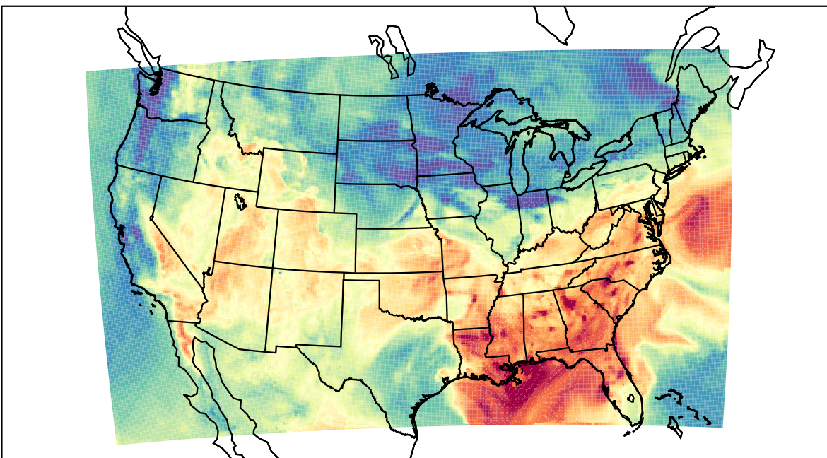
WRF (2019-09-08_17:00:00)
