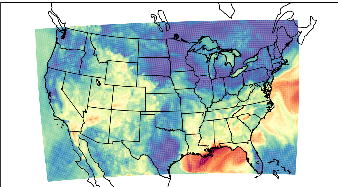
WRF (2019-09-09_07:00:00)
