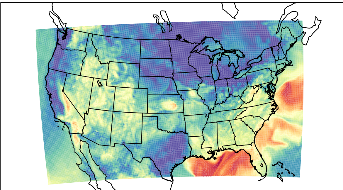
WRF (2019-09-08_14:00:00)
