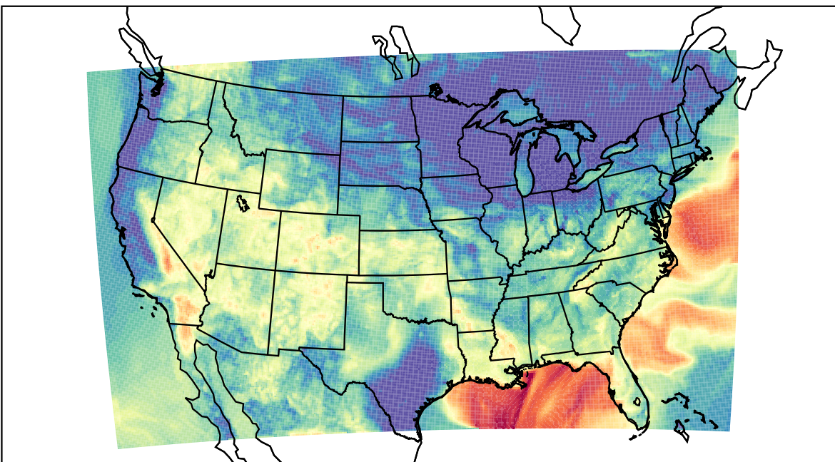
WRF (2019-09-08_08:00:00)
