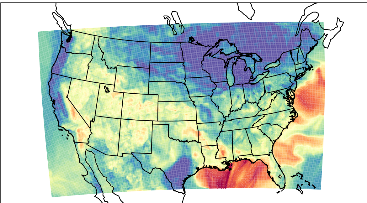
WRF (2019-09-08_06:00:00)
