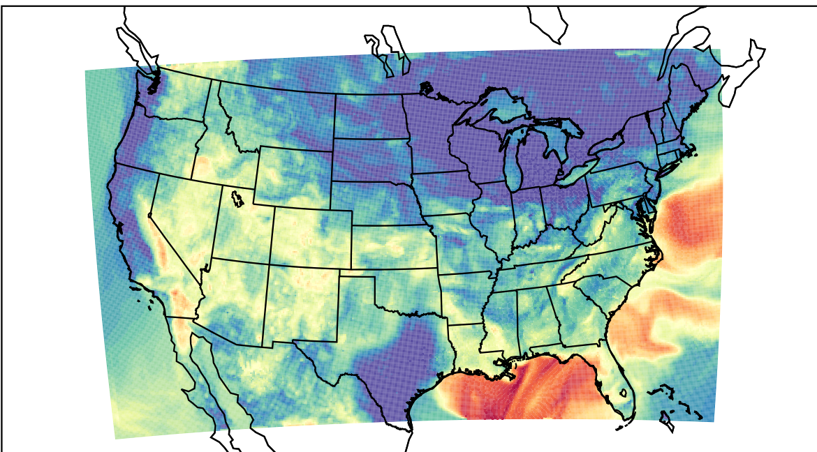
WRF (2019-09-08_10:00:00)
