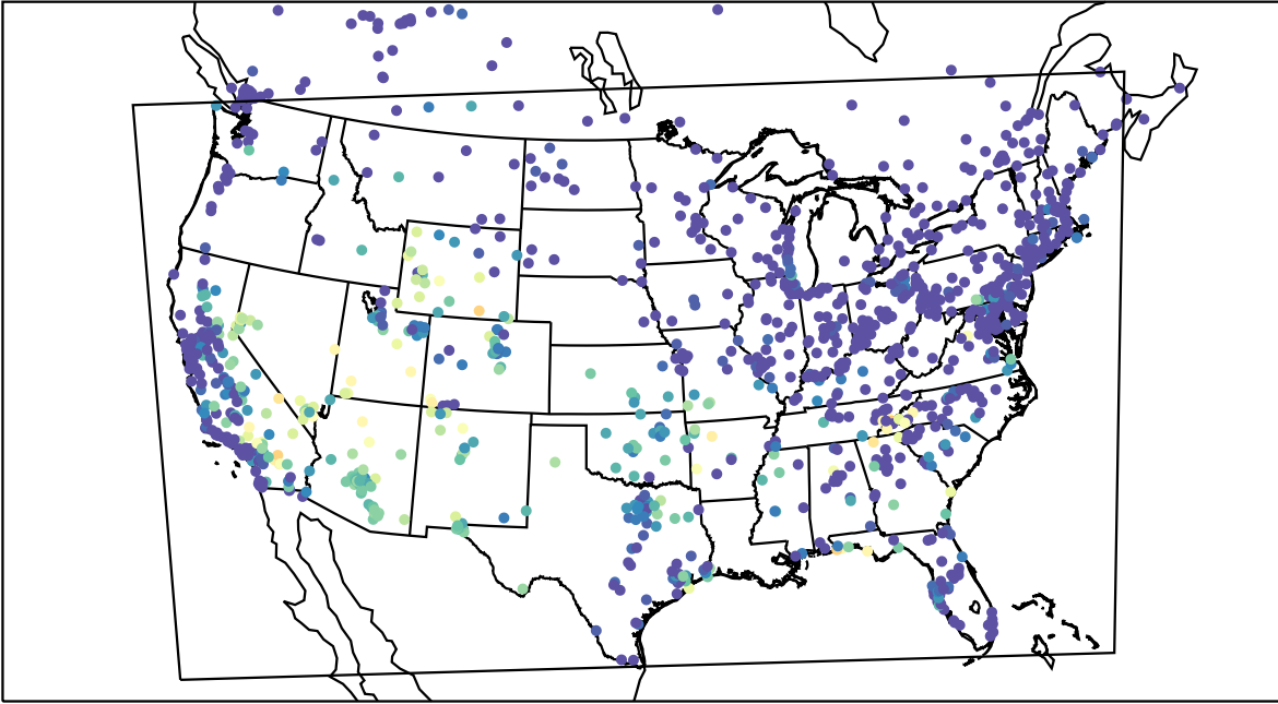
AirNOW (2019-09-09_07:00:00)
