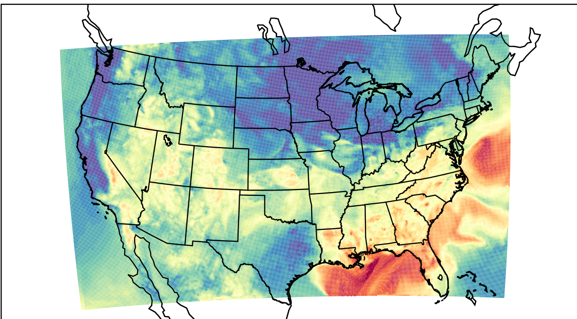
WRF (2019-09-08_15:00:00)
