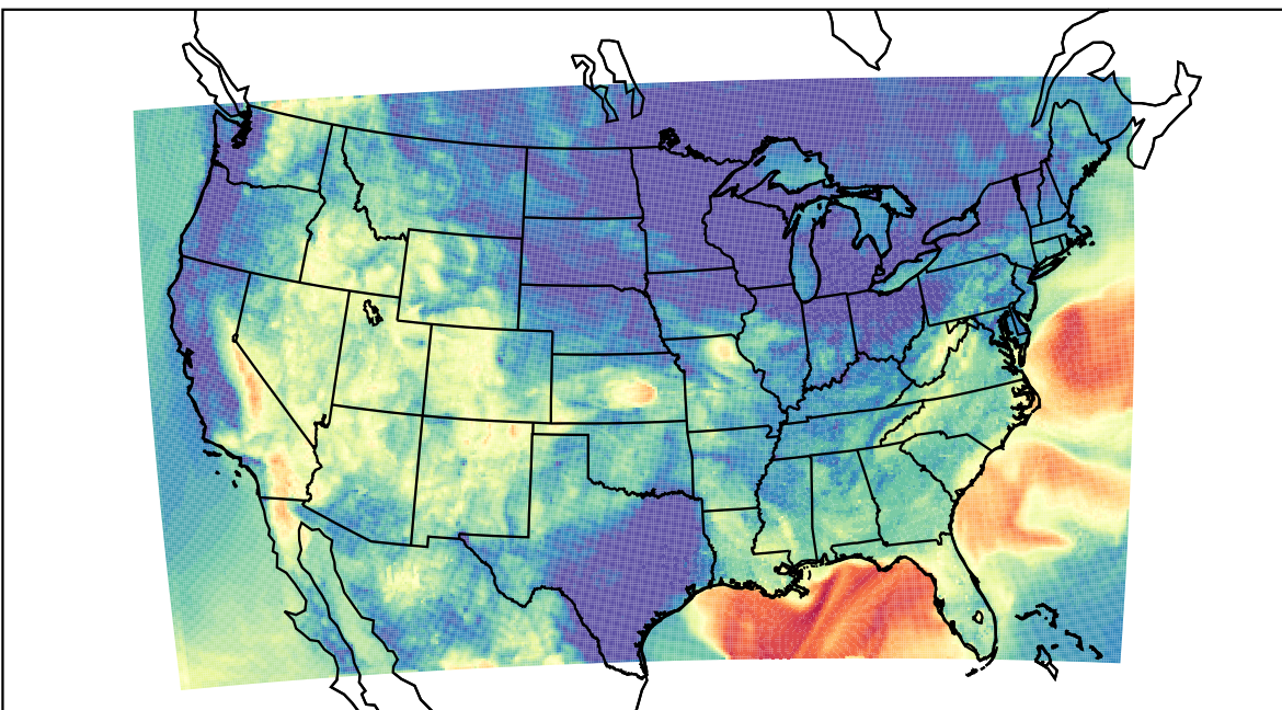
WRF (2019-09-08_13:00:00)
