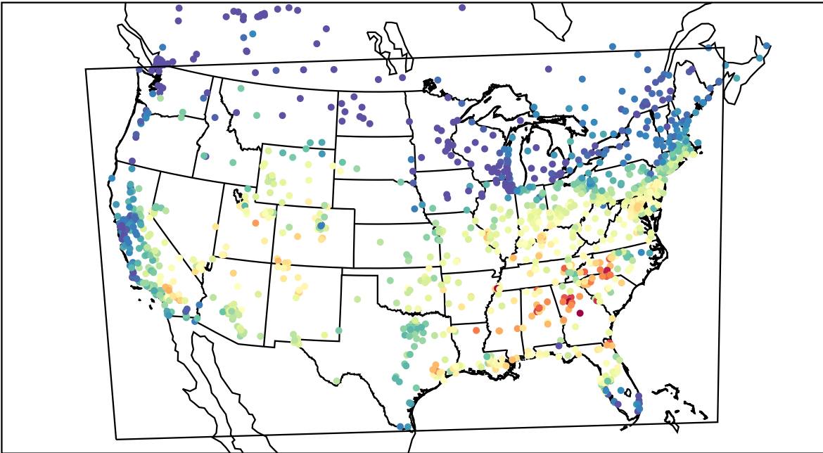
AirNOW (2019-09-09_17:00:00)
