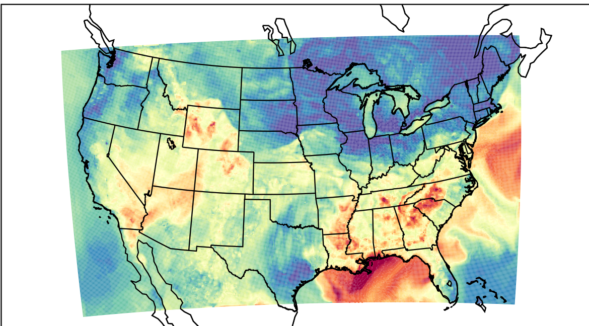
WRF (2019-09-09_02:00:00)
