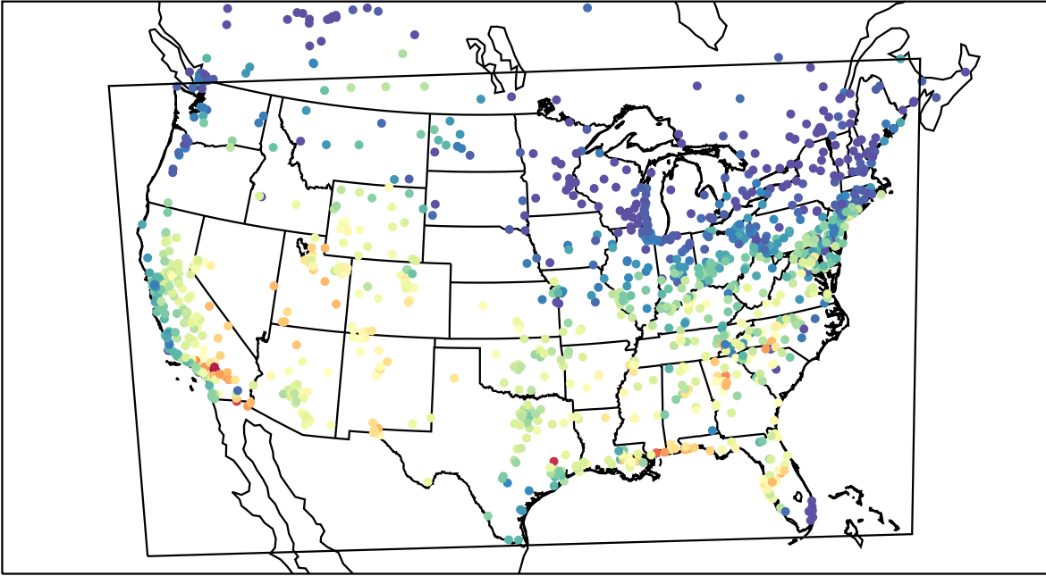
AirNOW (2019-09-08_23:00:00)
