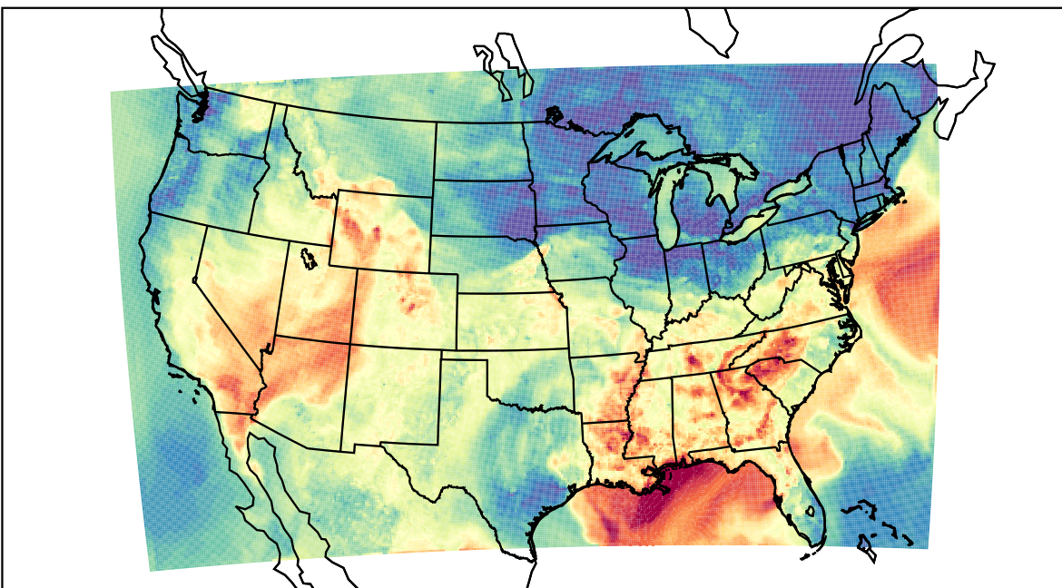
WRF (2019-09-09_01:00:00)
