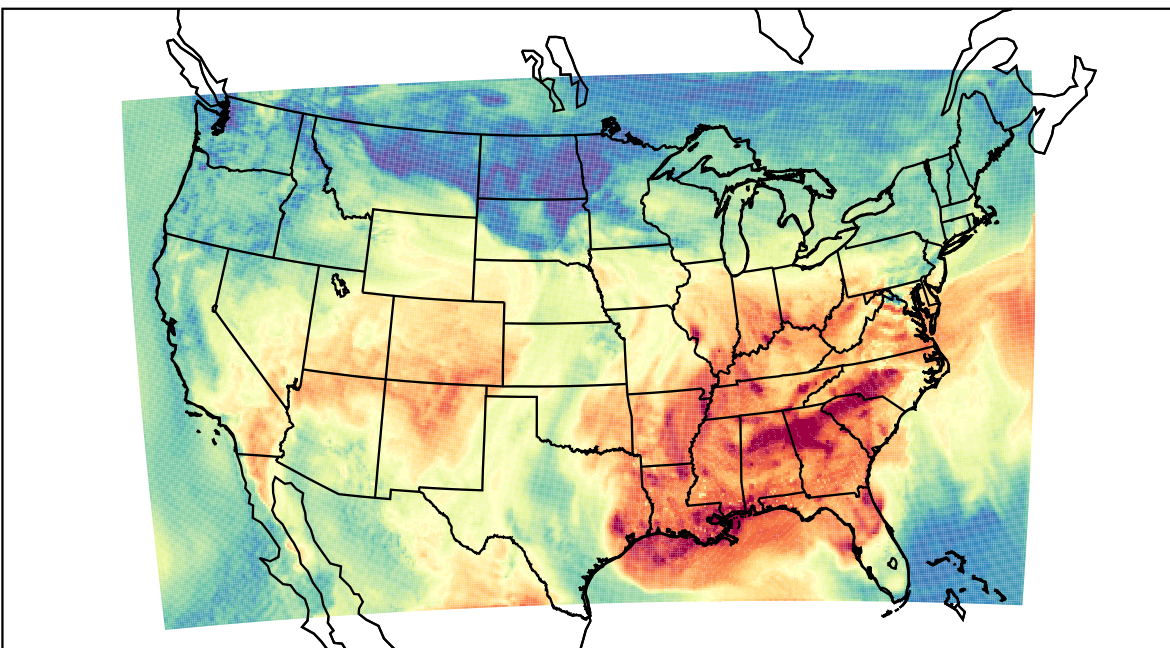
WRF (2019-09-09_18:00:00)
