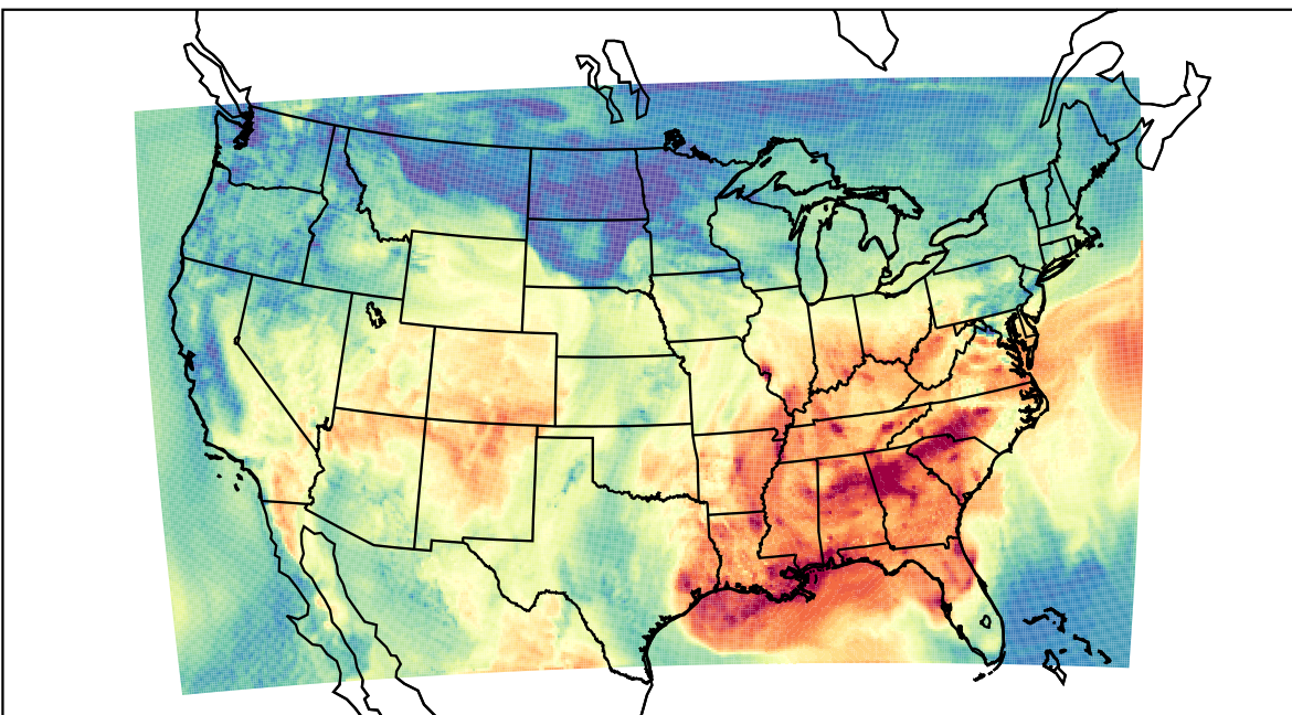
WRF (2019-09-09_17:00:00)
