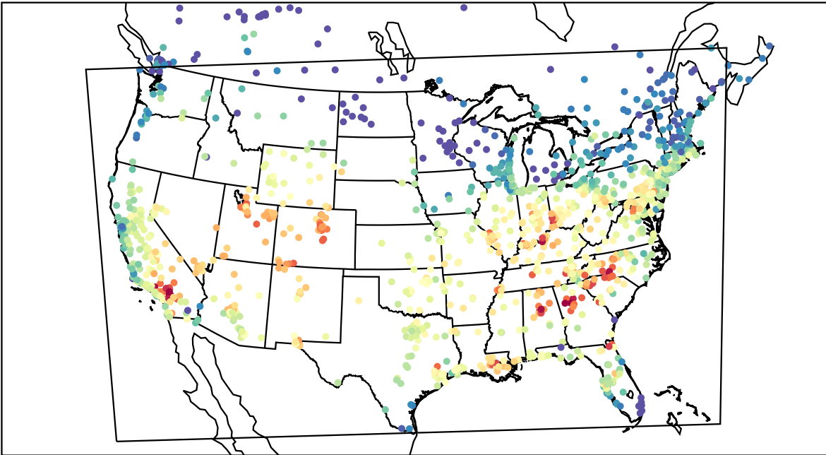
AirNOW (2019-09-09_21:00:00)
