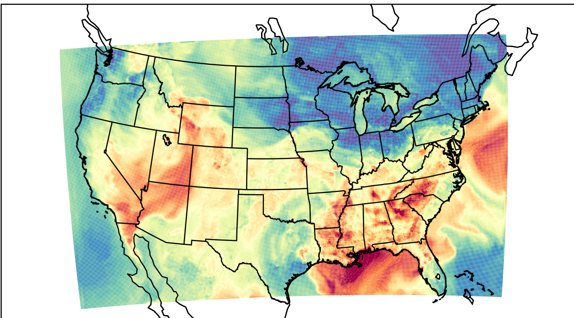
WRF (2019-09-09_00:00:00)
