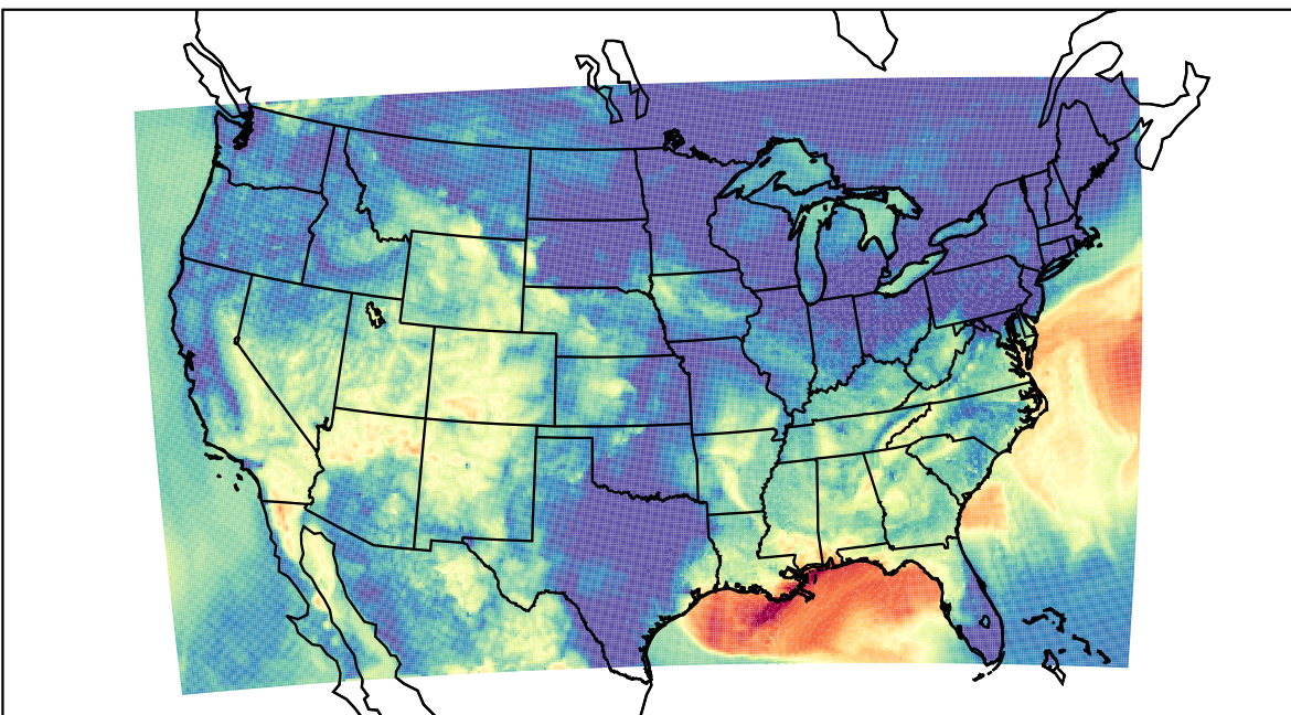
WRF (2019-09-09_12:00:00)
