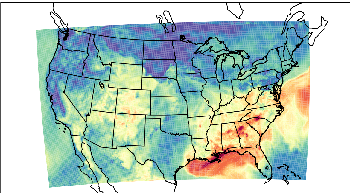
WRF (2019-09-09_15:00:00)
