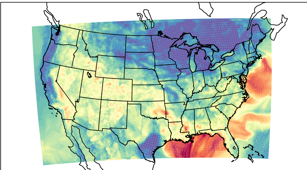
WRF (2019-09-08_05:00:00)
