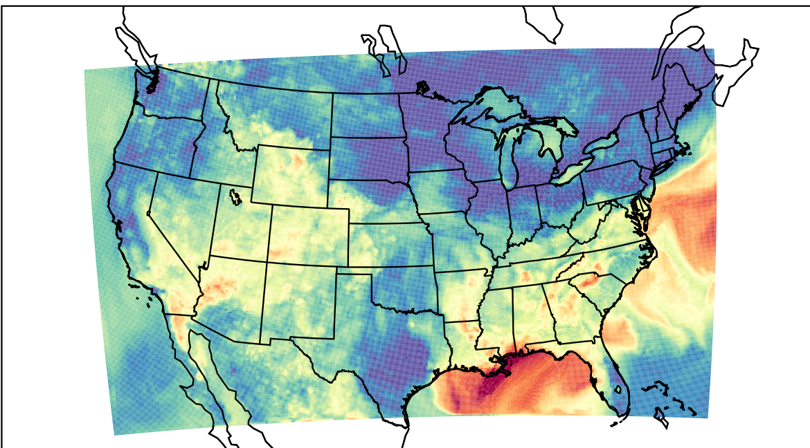
WRF (2019-09-09_06:00:00)
