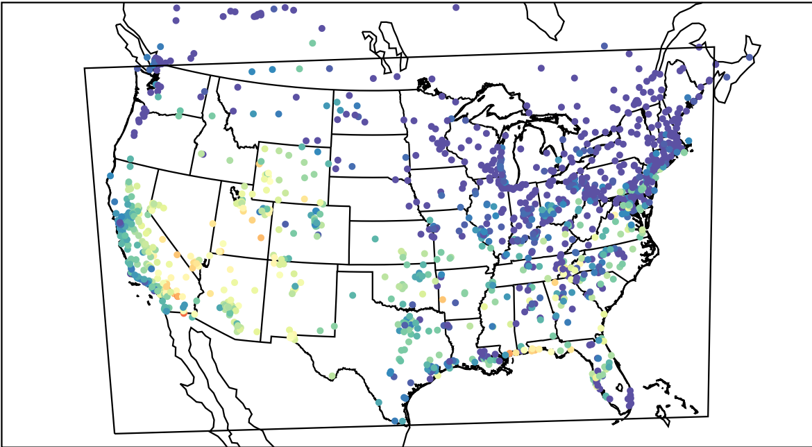
AirNOW (2019-09-09_02:00:00)
