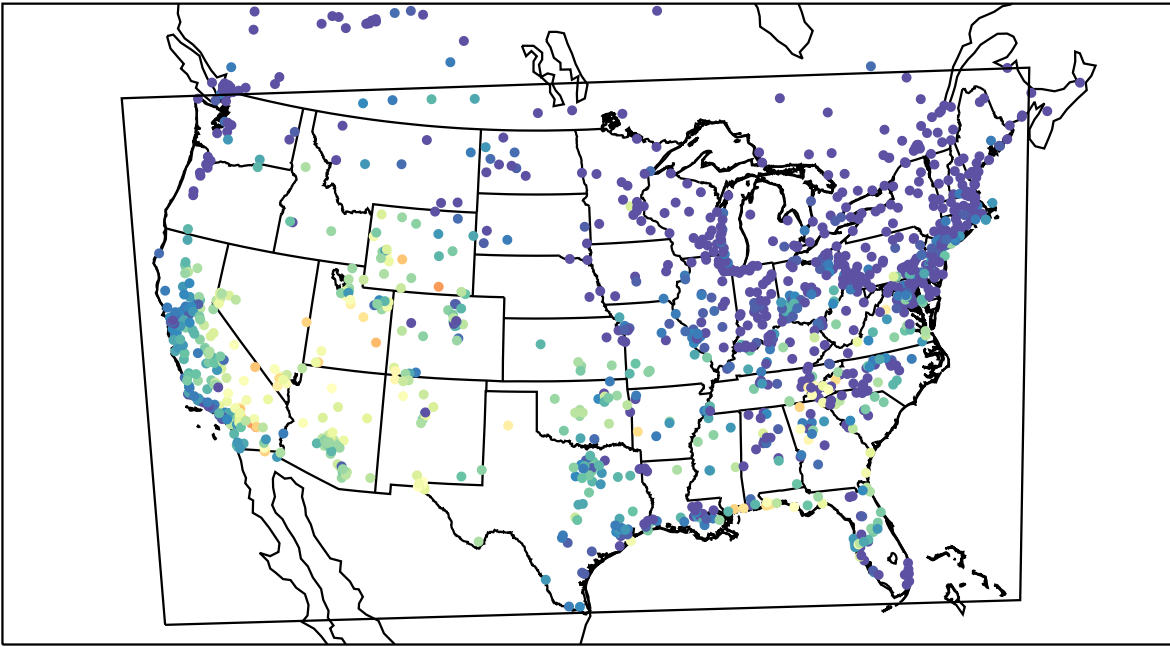
AirNOW (2019-09-09_03:00:00)
