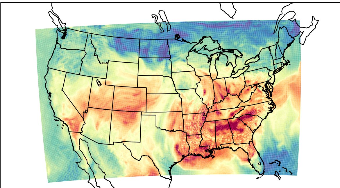
WRF (2019-09-09_22:00:00)
