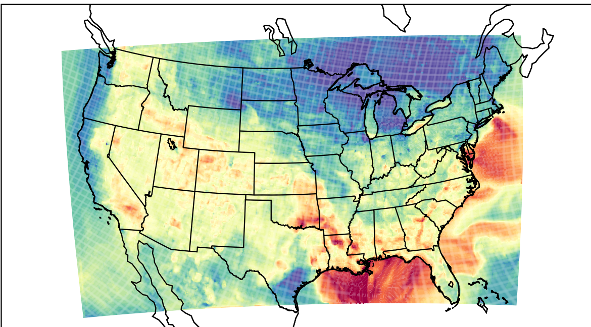
WRF (2019-09-08_02:00:00)
