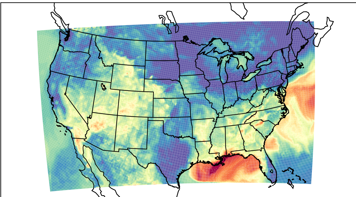
WRF (2019-09-09_08:00:00)
