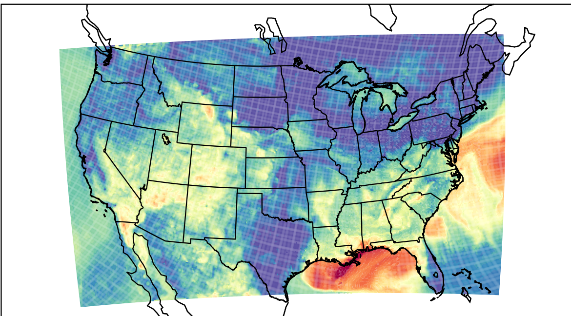
WRF (2019-09-09_10:00:00)
