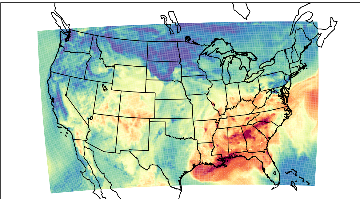
WRF (2019-09-09_16:00:00)
