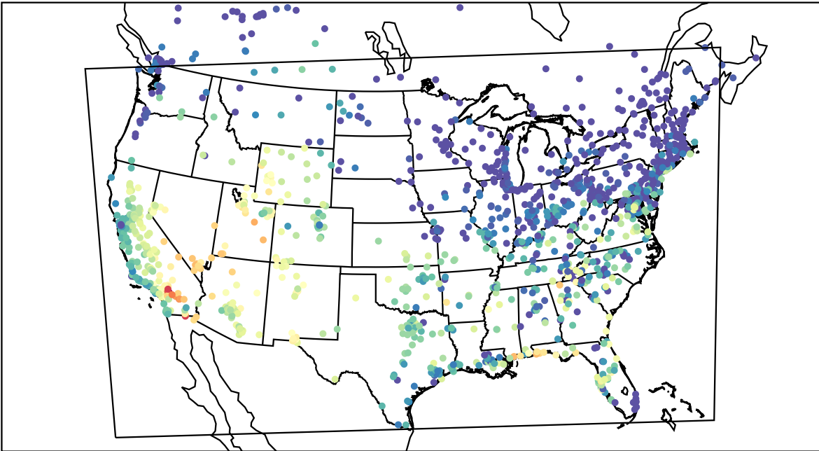
AirNOW (2019-09-09_01:00:00)
