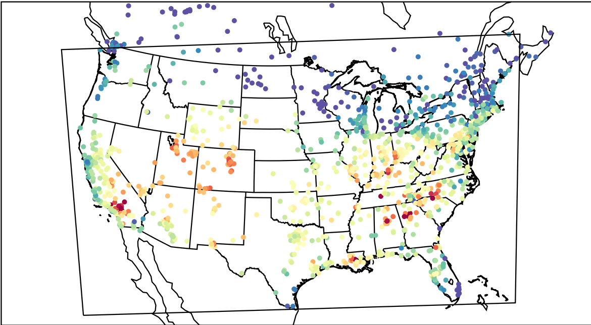
AirNOW (2019-09-09_22:00:00)
