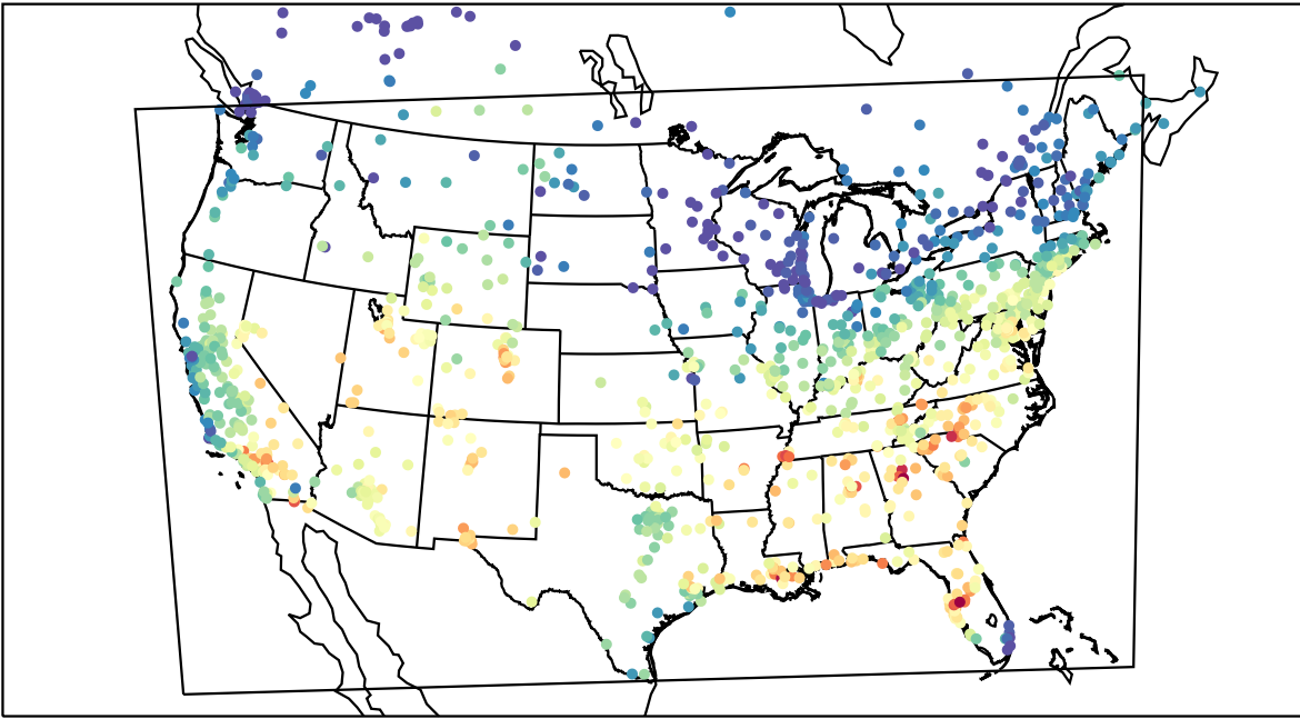
AirNOW (2019-09-08_20:00:00)
