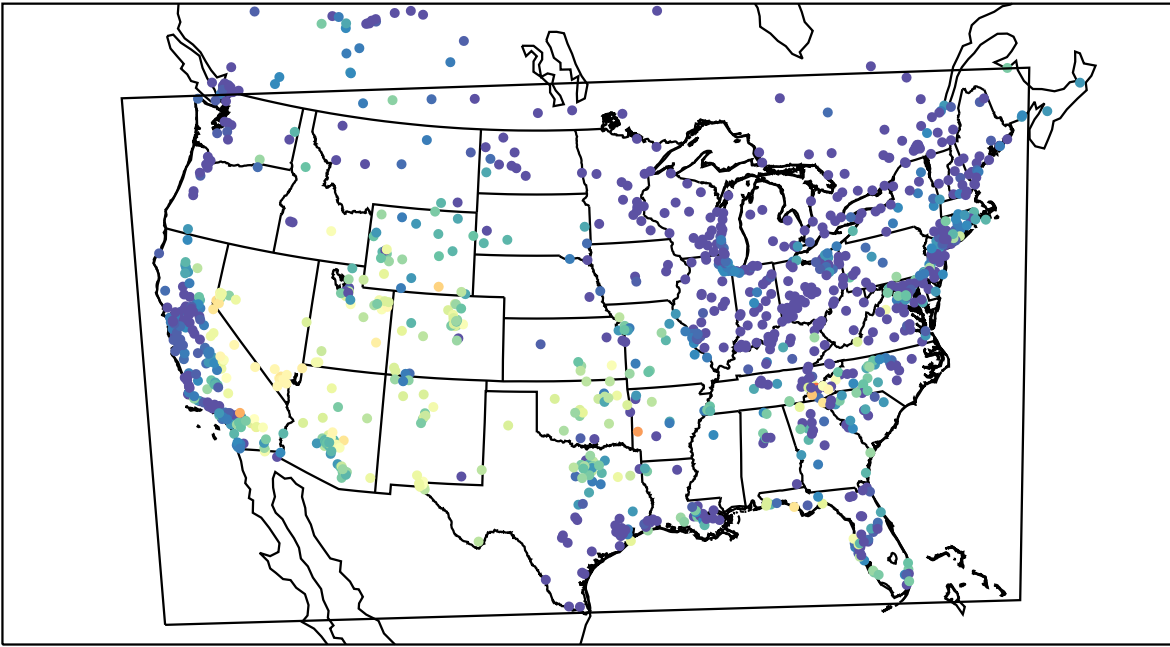
AirNOW (2019-09-08_06:00:00)
