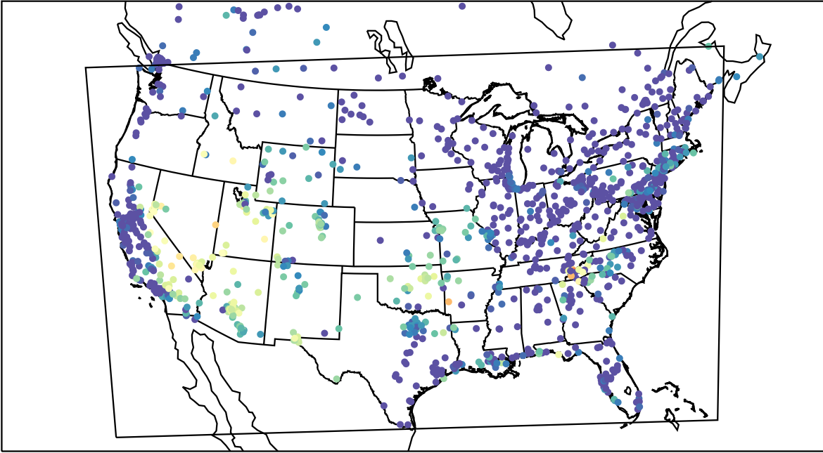
AirNOW (2019-09-08_09:00:00)
