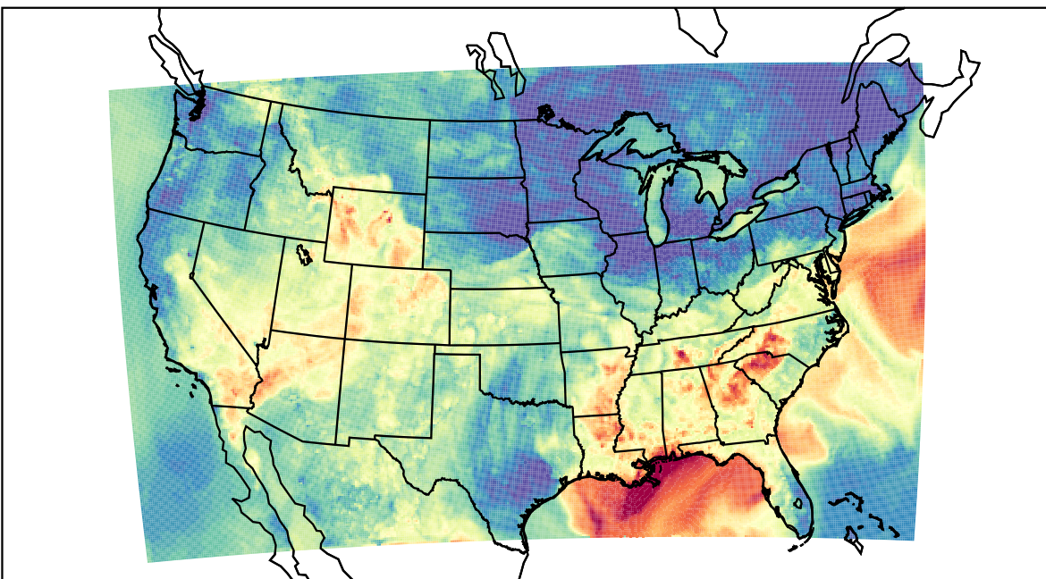
WRF (2019-09-09_03:00:00)
