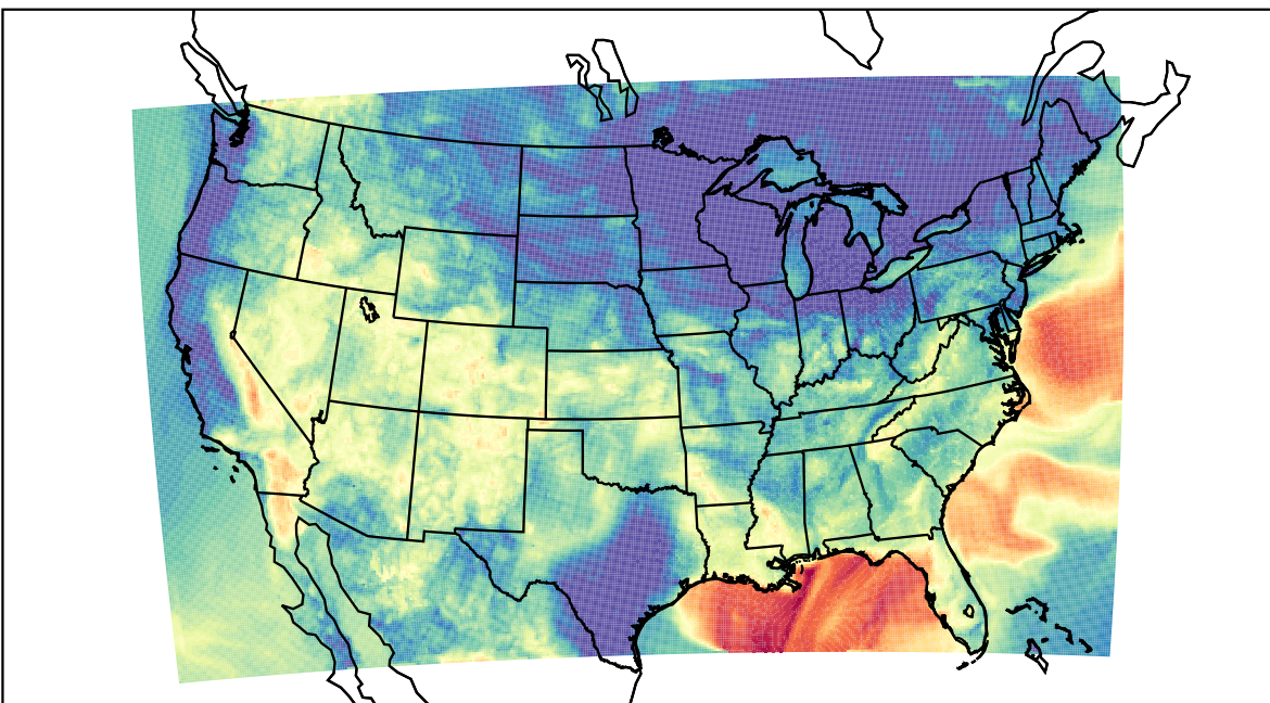
WRF (2019-09-08_09:00:00)
