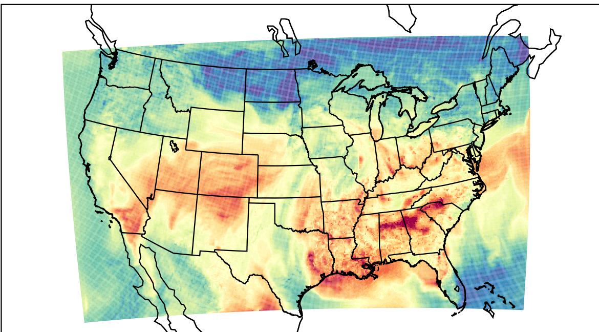
WRF (2019-09-09_23:00:00)
