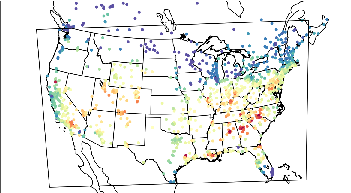
AirNOW (2019-09-09_19:00:00)
