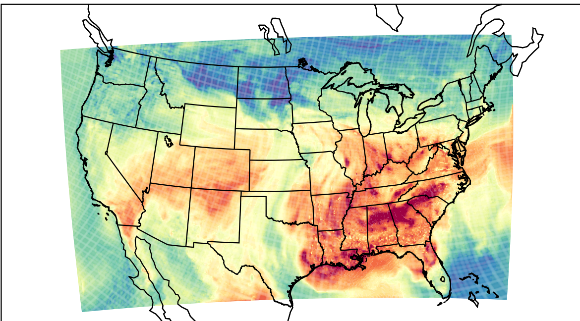
WRF (2019-09-09_20:00:00)
