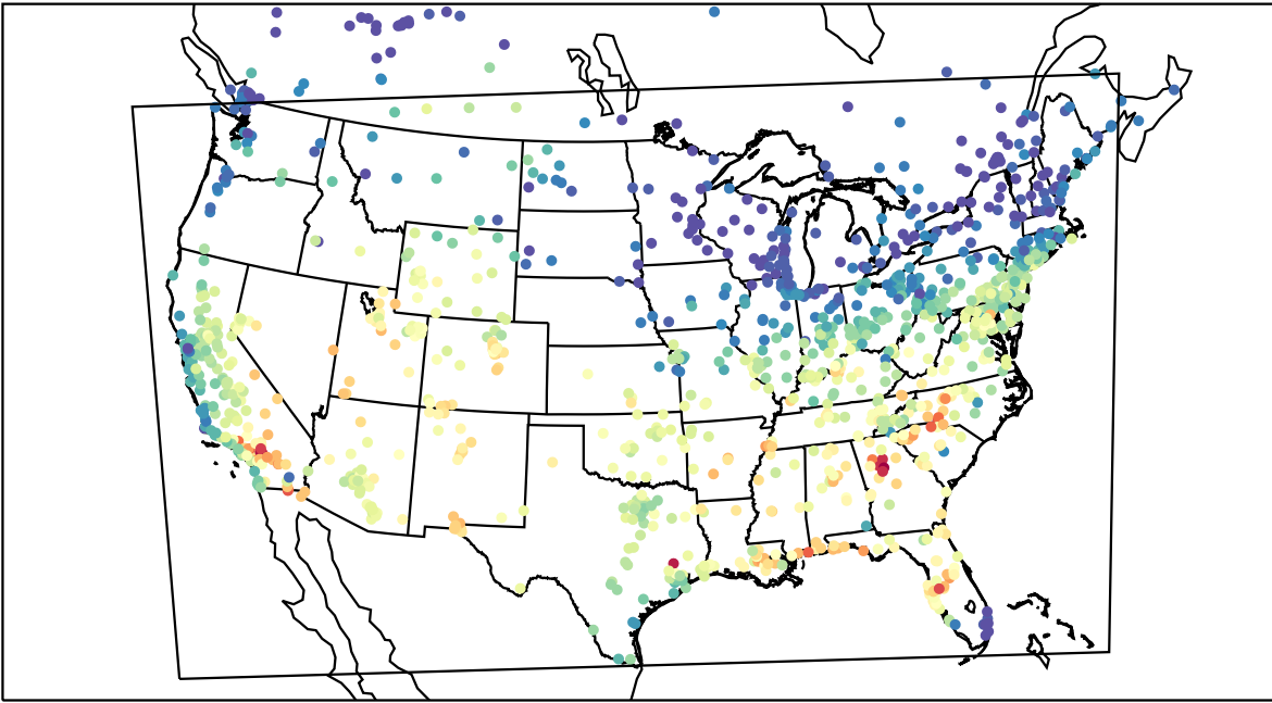
AirNOW (2019-09-08_22:00:00)
