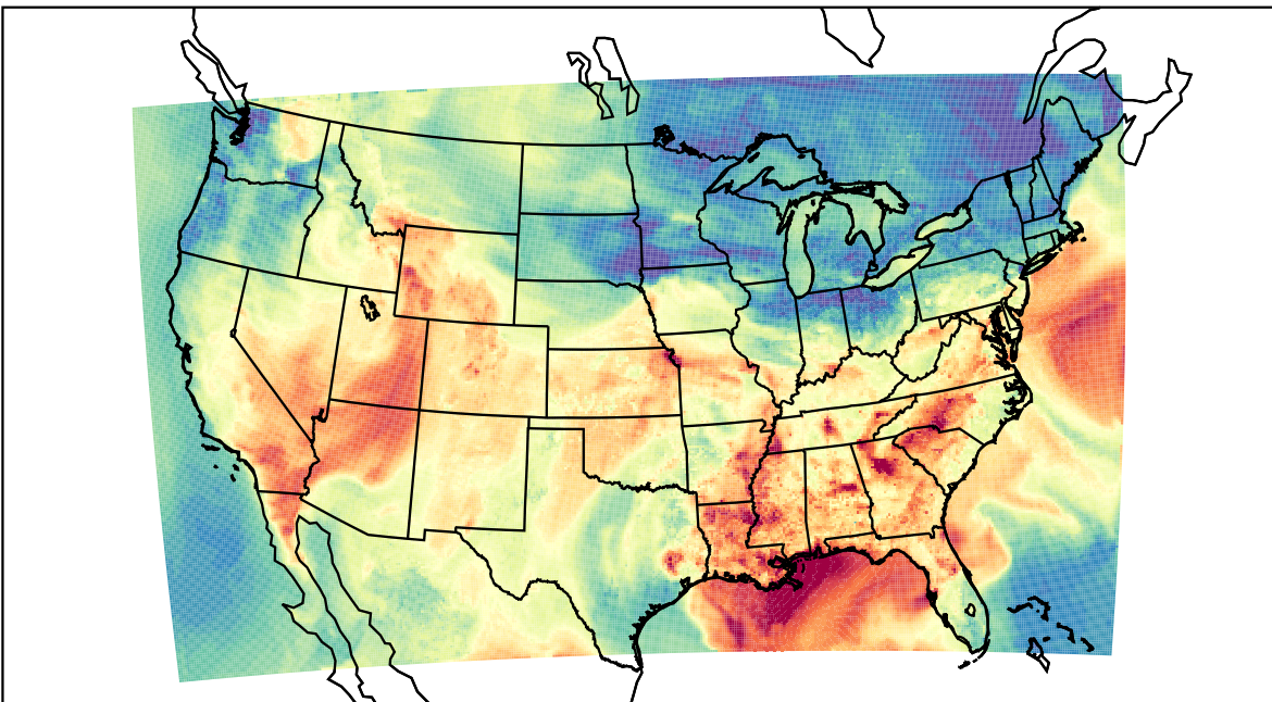
WRF (2019-09-08_23:00:00)
