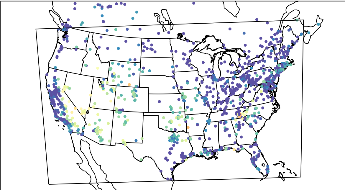
AirNOW (2019-09-08_08:00:00)
