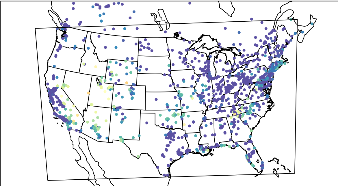
AirNOW (2019-09-08_12:00:00)
