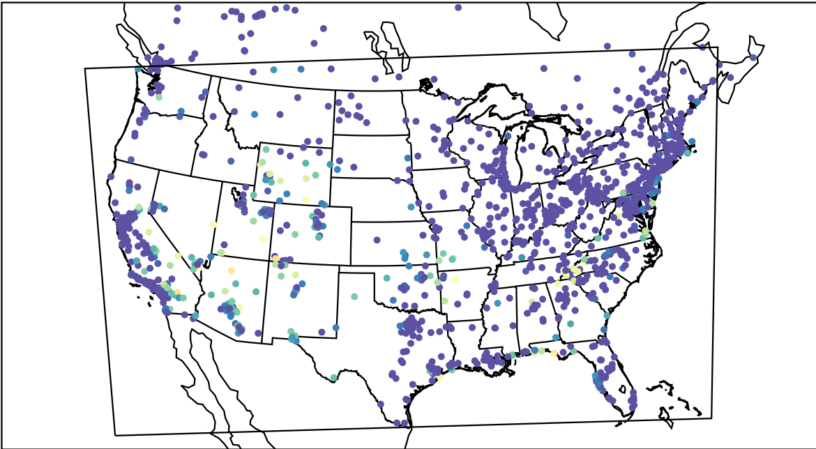
AirNOW (2019-09-09_12:00:00)
