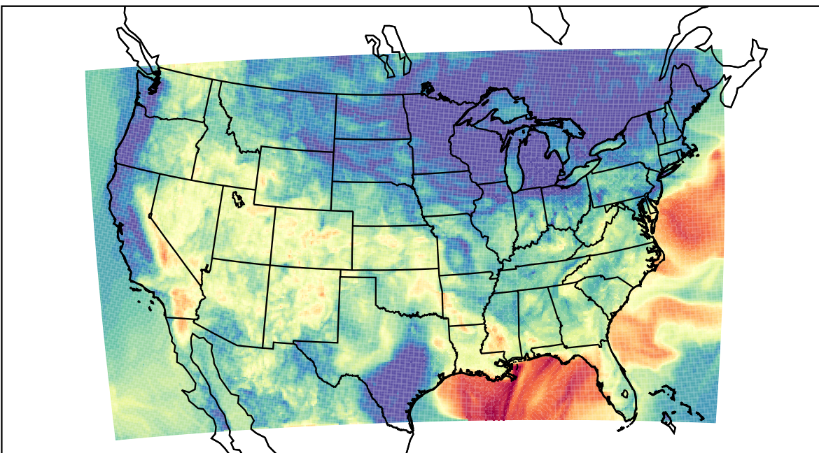
WRF (2019-09-08_07:00:00)
