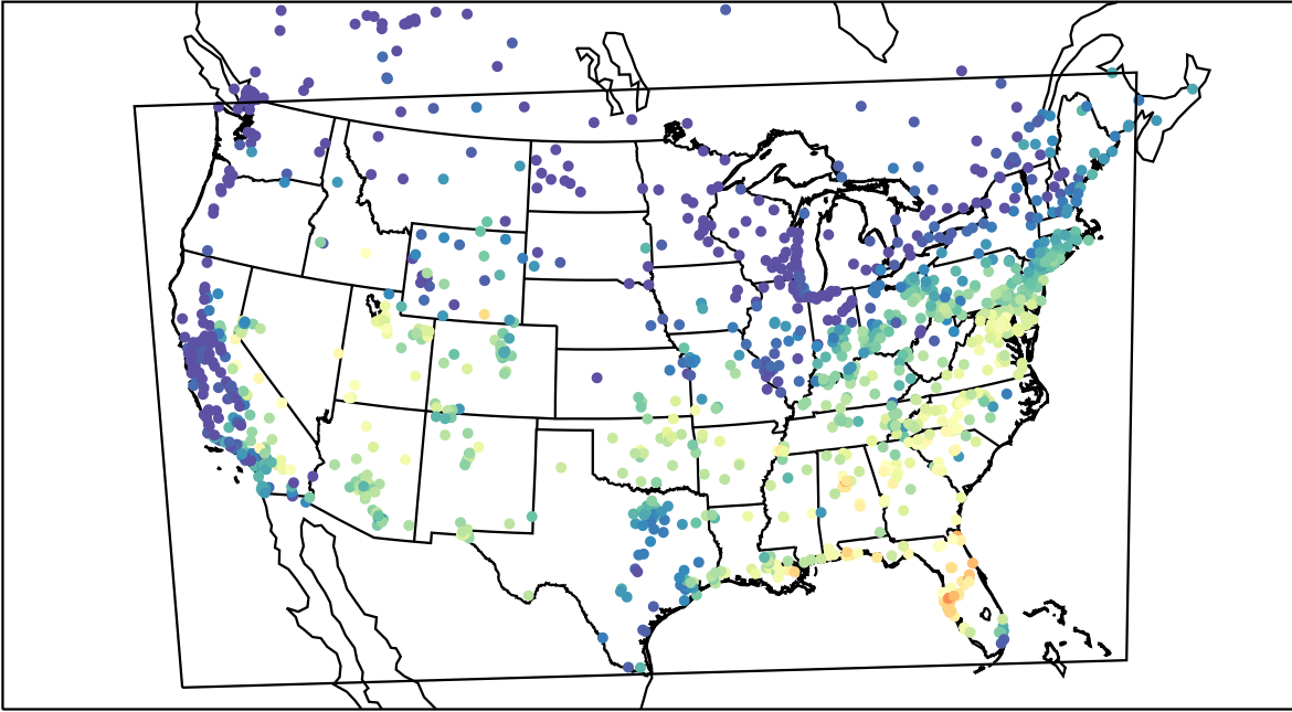
AirNOW (2019-09-08_15:00:00)
