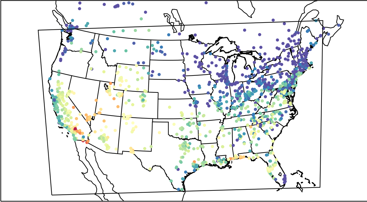
AirNOW (2019-09-09_00:00:00)
