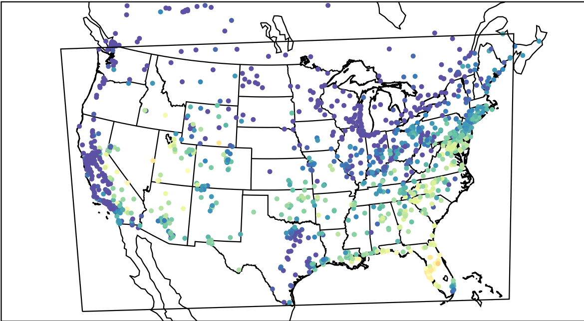
AirNOW (2019-09-08_14:00:00)
