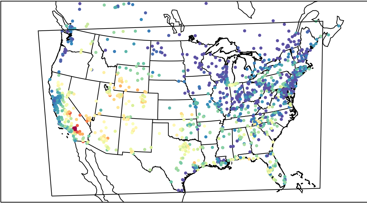
AirNOW (2019-09-08_01:00:00)
