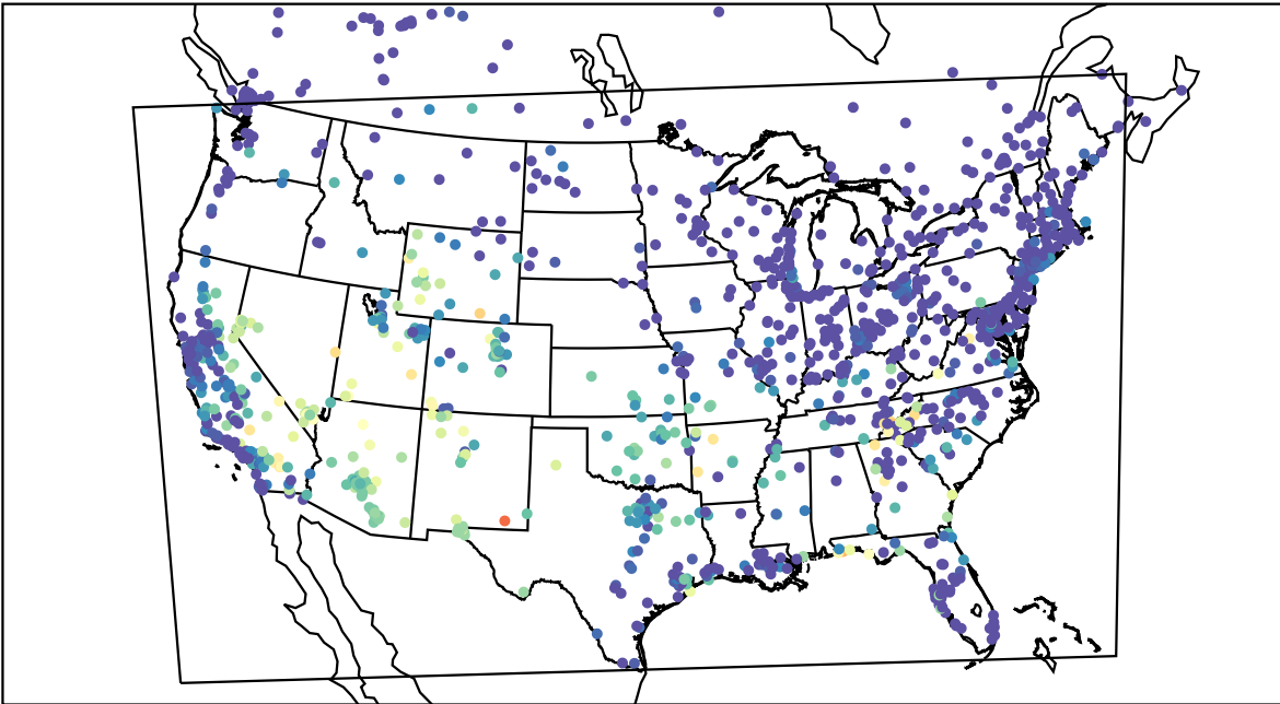
AirNOW (2019-09-09_06:00:00)
