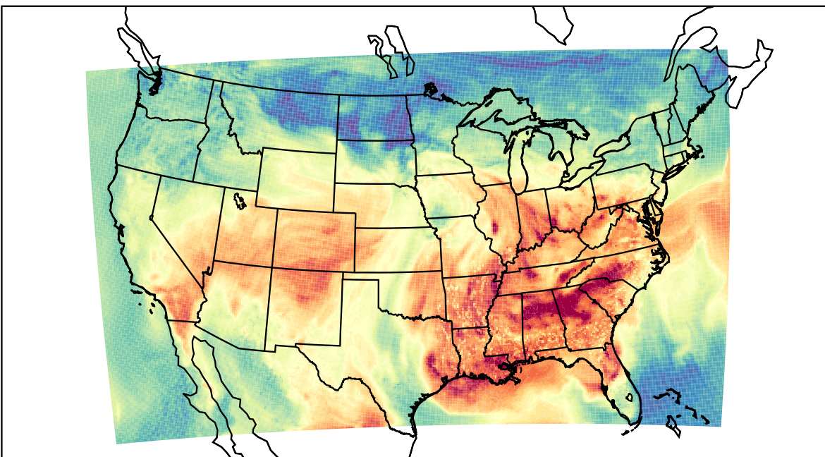
WRF (2019-09-09_21:00:00)
