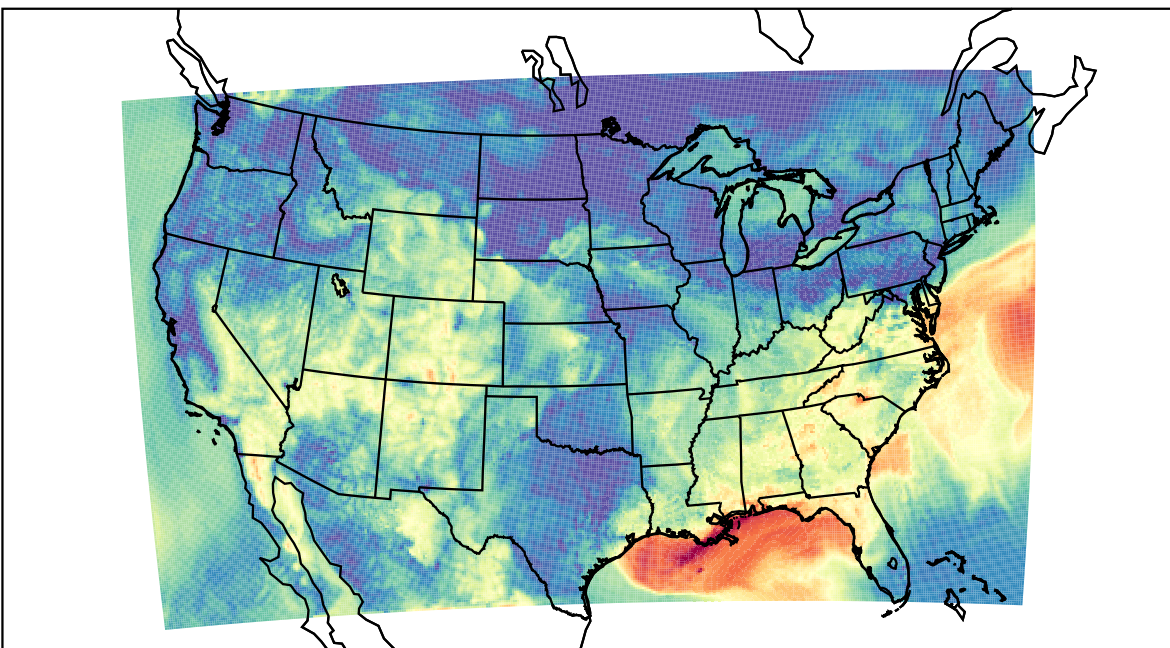
WRF (2019-09-09_14:00:00)
