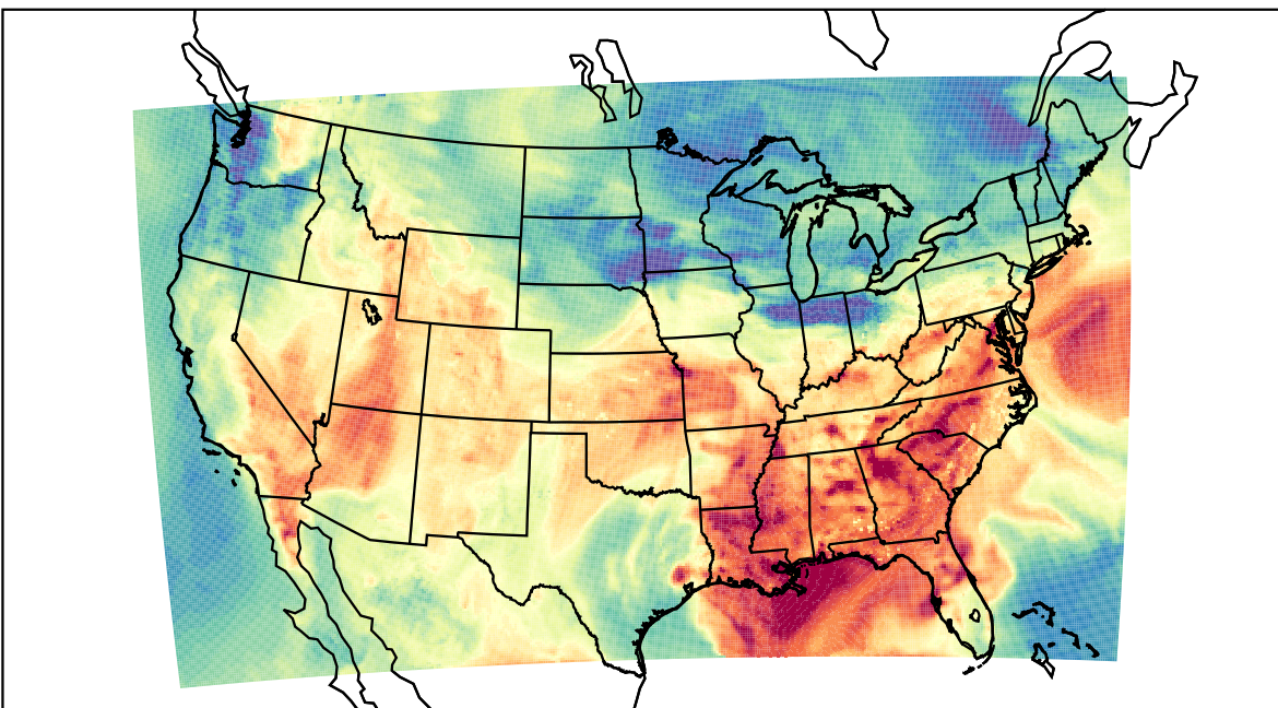
WRF (2019-09-08_20:00:00)
