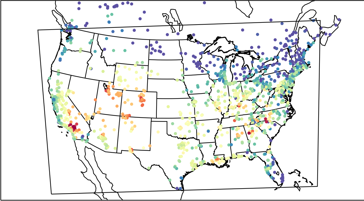
AirNOW (2019-09-09_23:00:00)
