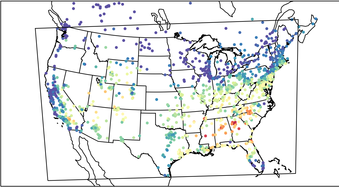
AirNOW (2019-09-09_16:00:00)
