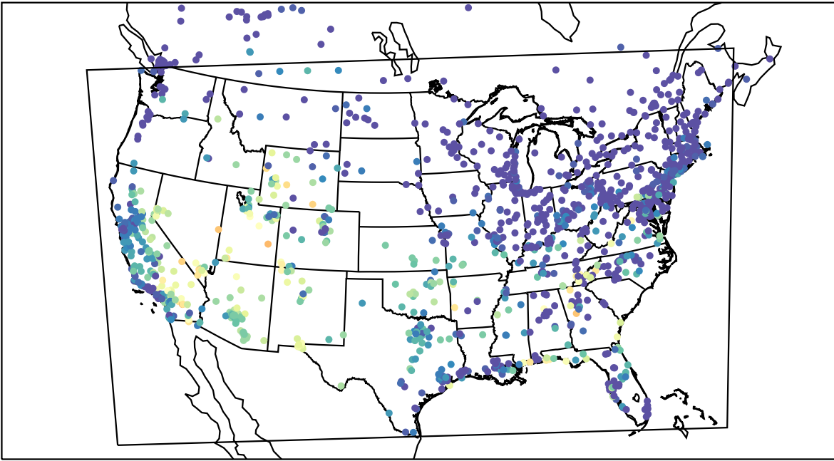
AirNOW (2019-09-09_04:00:00)
