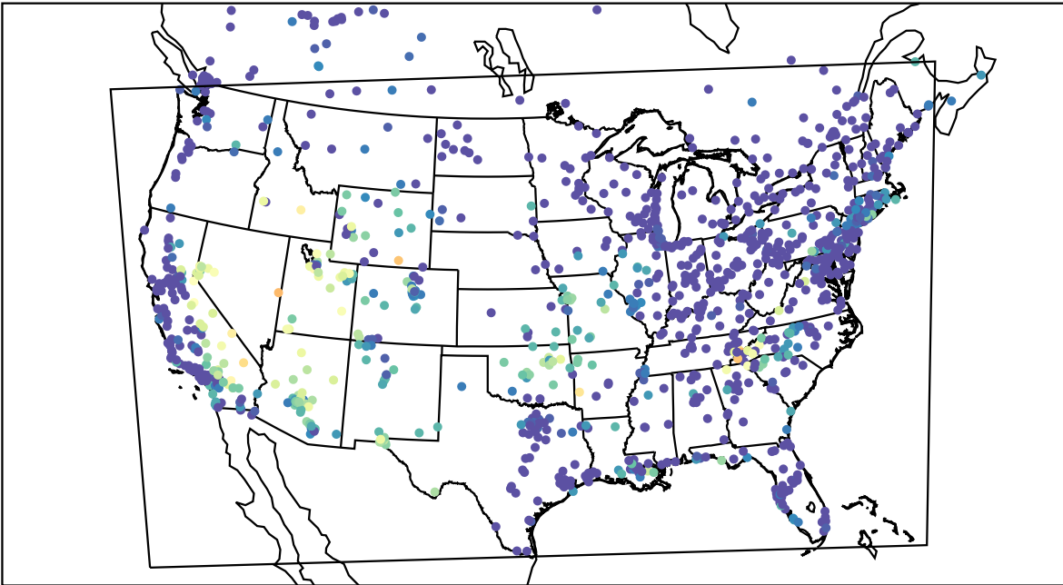
AirNOW (2019-09-08_11:00:00)
