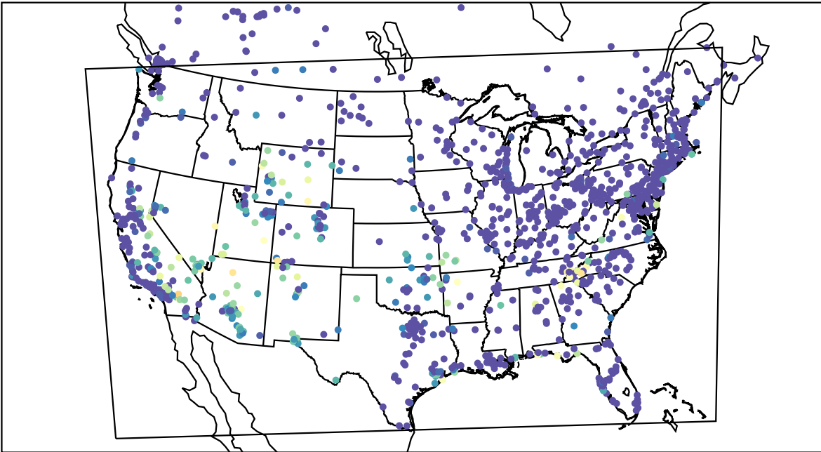
AirNOW (2019-09-09_11:00:00)
