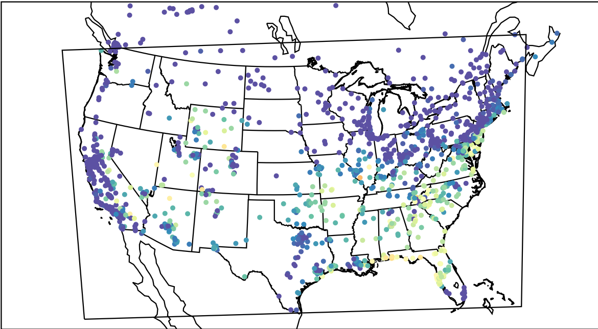
AirNOW (2019-09-09_14:00:00)
