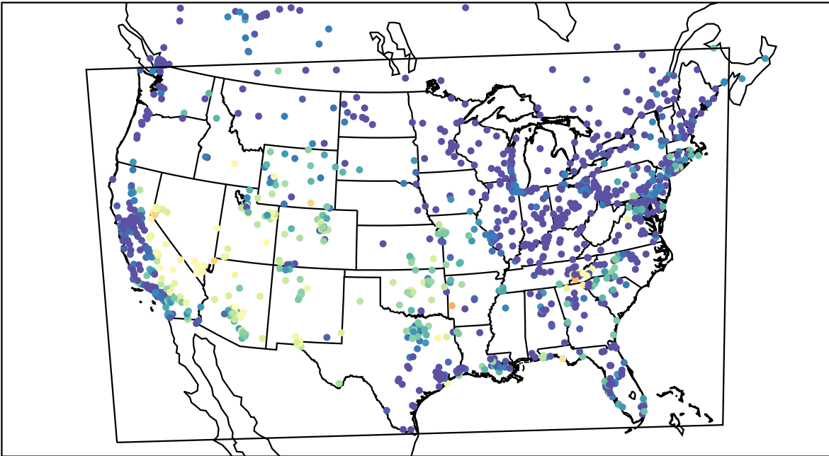
AirNOW (2019-09-08_07:00:00)
