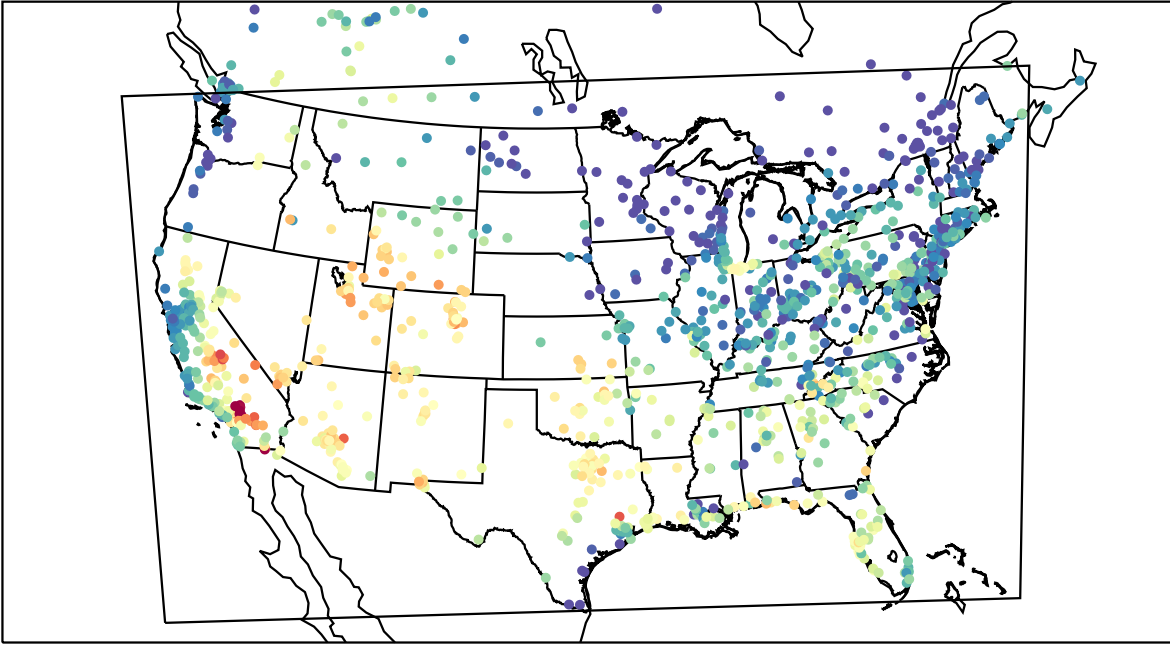
AirNOW (2019-09-08_00:00:00)
