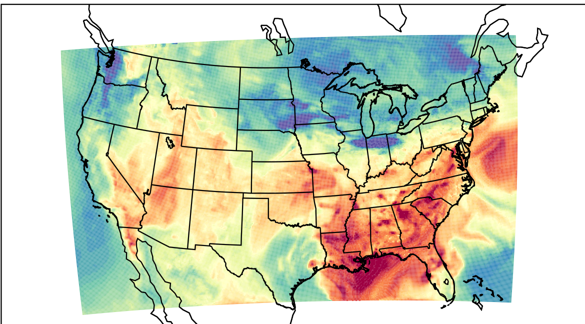
WRF (2019-09-08_19:00:00)
