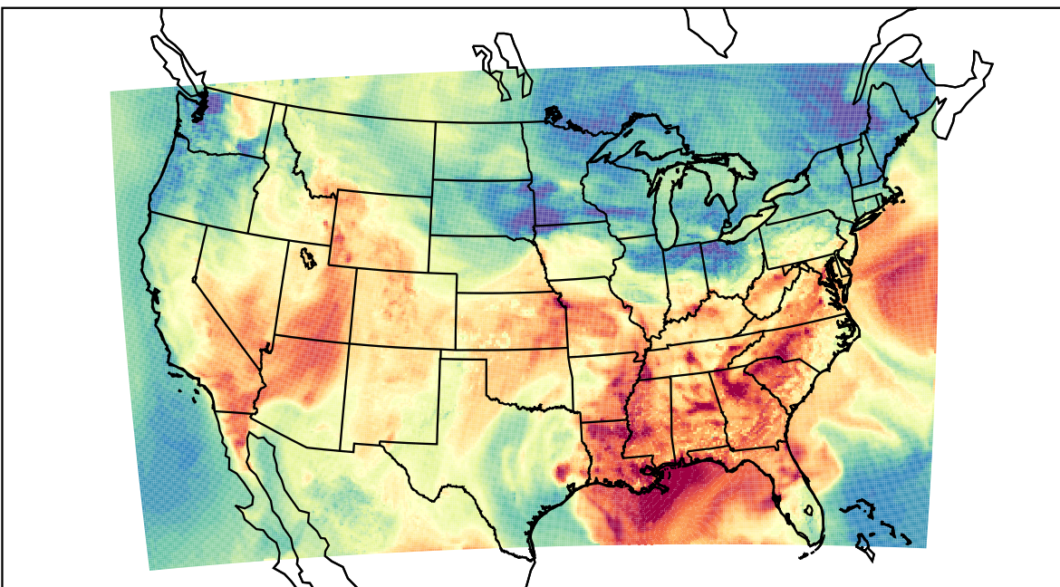
WRF (2019-09-08_22:00:00)
