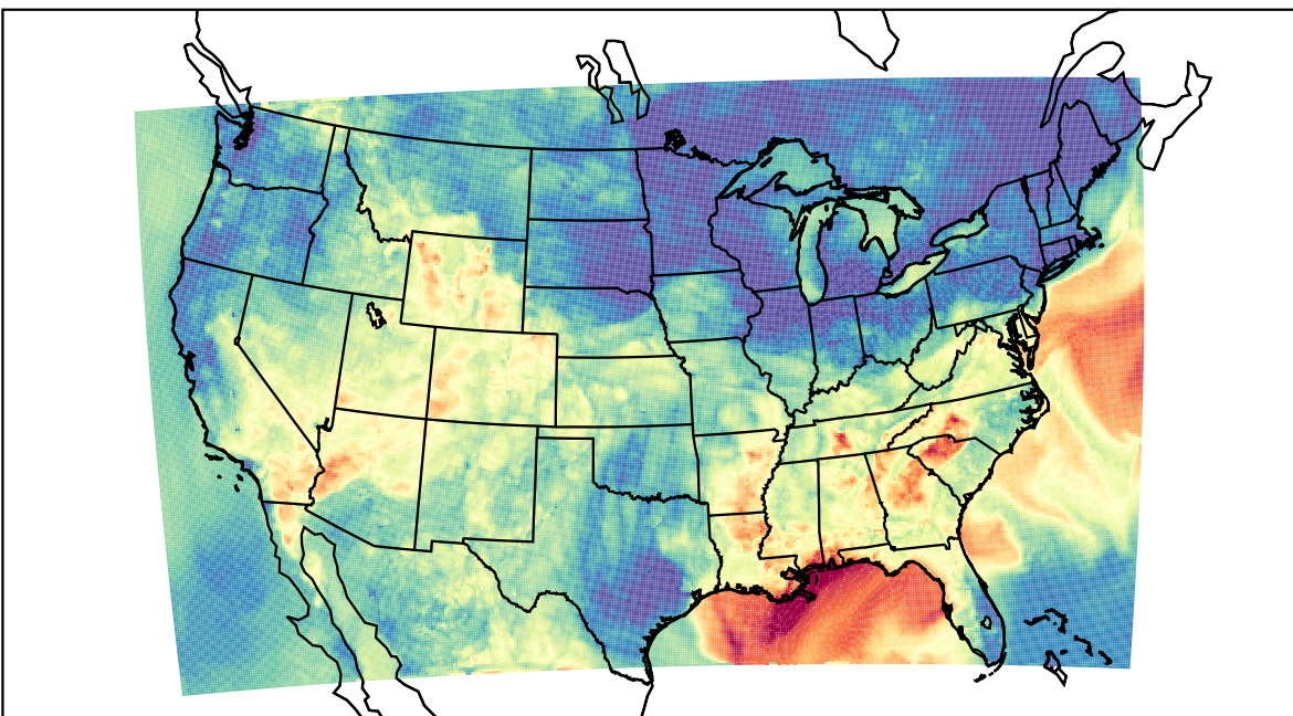
WRF (2019-09-09_04:00:00)
