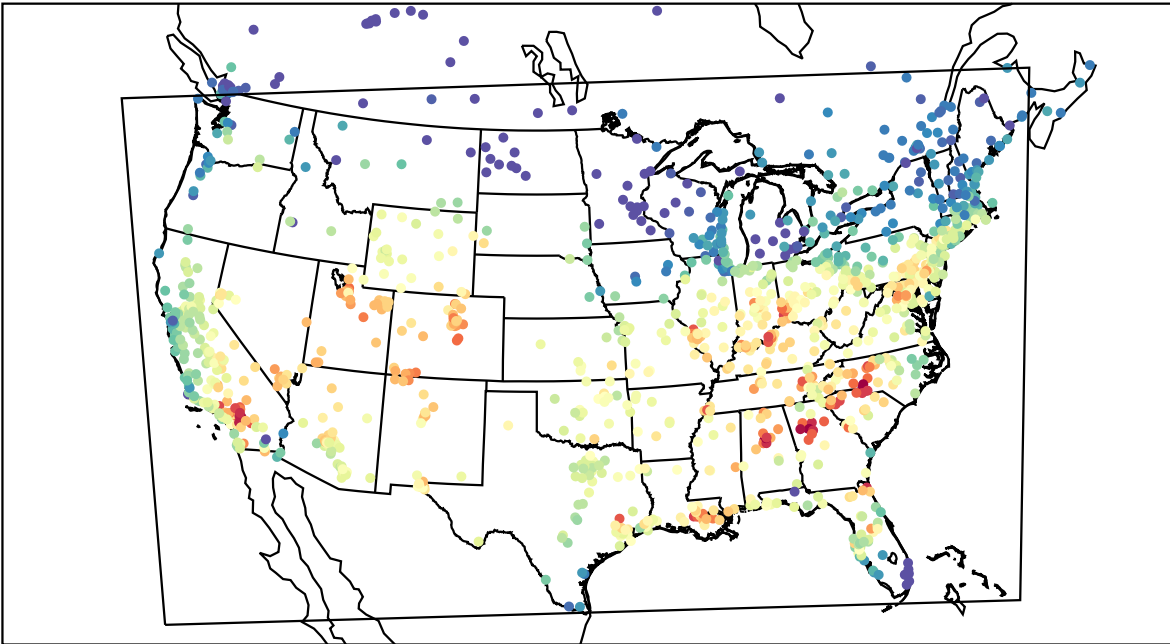
AirNOW (2019-09-09_20:00:00)
