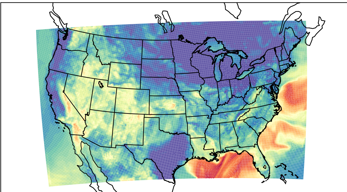
WRF (2019-09-08_12:00:00)
