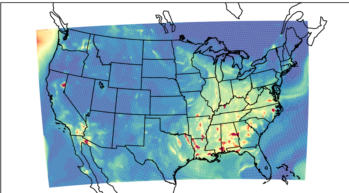
WRF 2019-09-13_06:00:00
