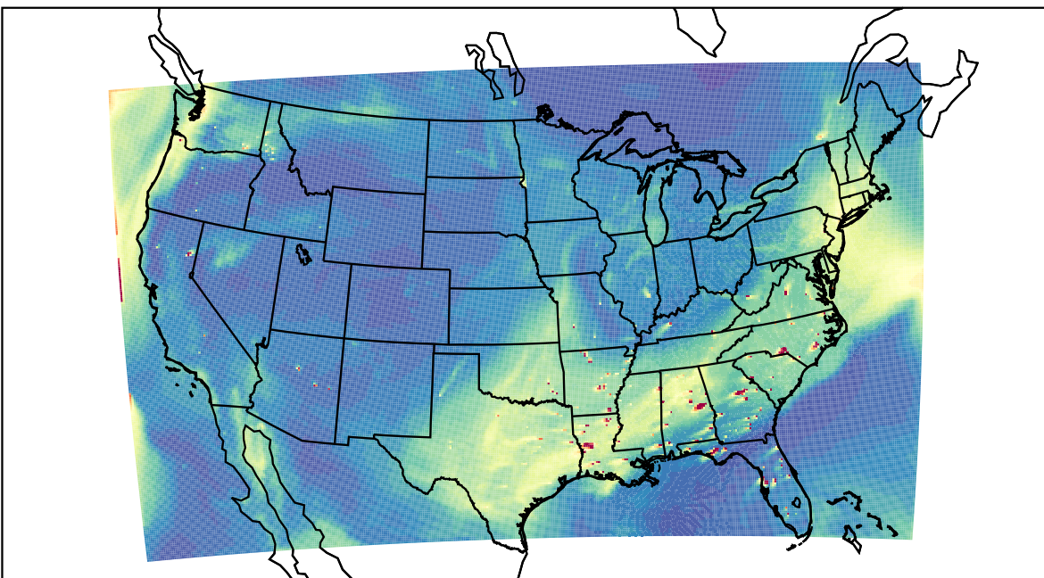
WRF 2019-09-14_21:00:00
