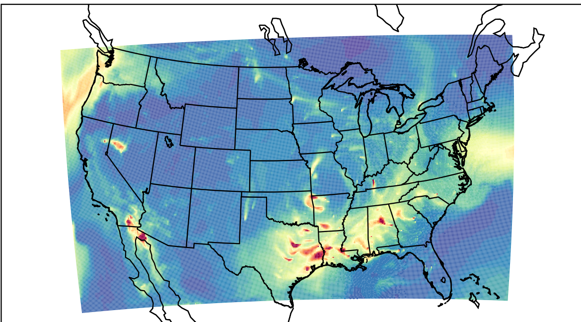
WRF 2019-09-14_09:00:00
