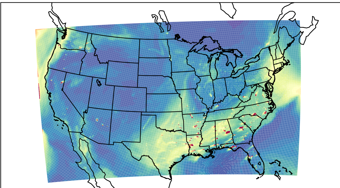
WRF 2019-09-14_22:00:00
