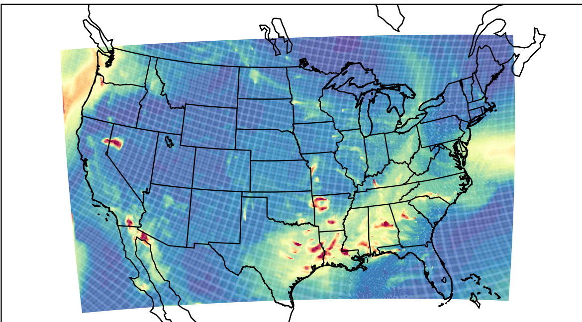
WRF 2019-09-14_06:00:00
