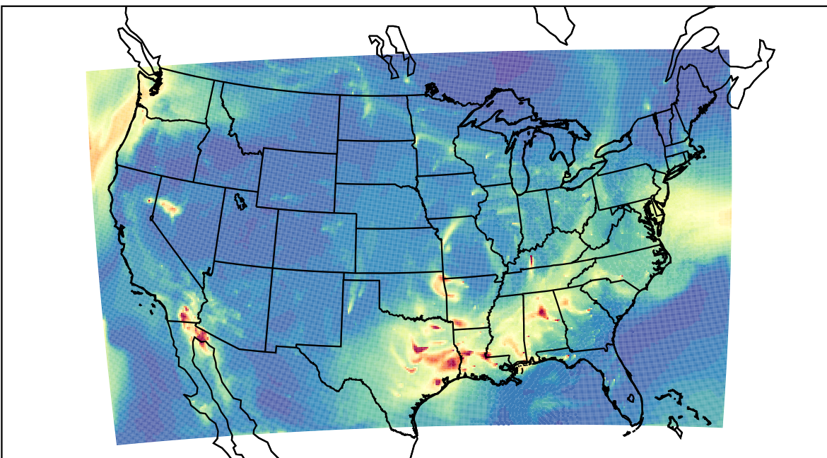
WRF 2019-09-14_10:00:00
