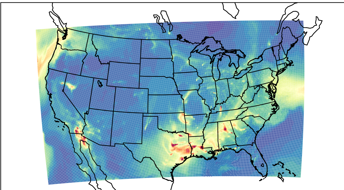
WRF 2019-09-14_11:00:00
