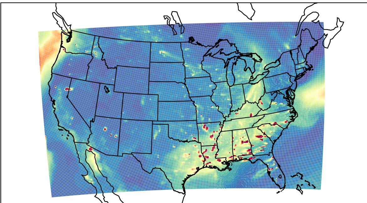
WRF 2019-09-14_01:00:00
