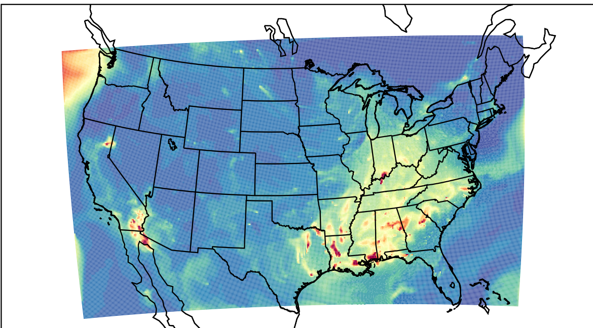
WRF 2019-09-13_11:00:00
