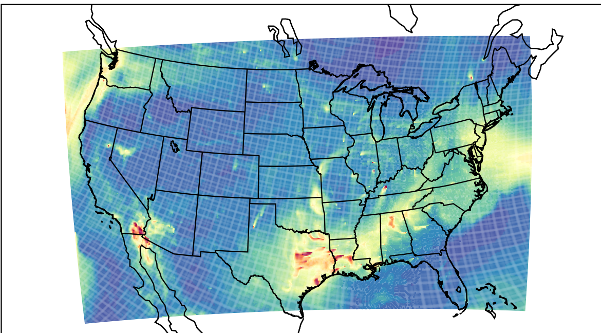
WRF 2019-09-14_14:00:00
