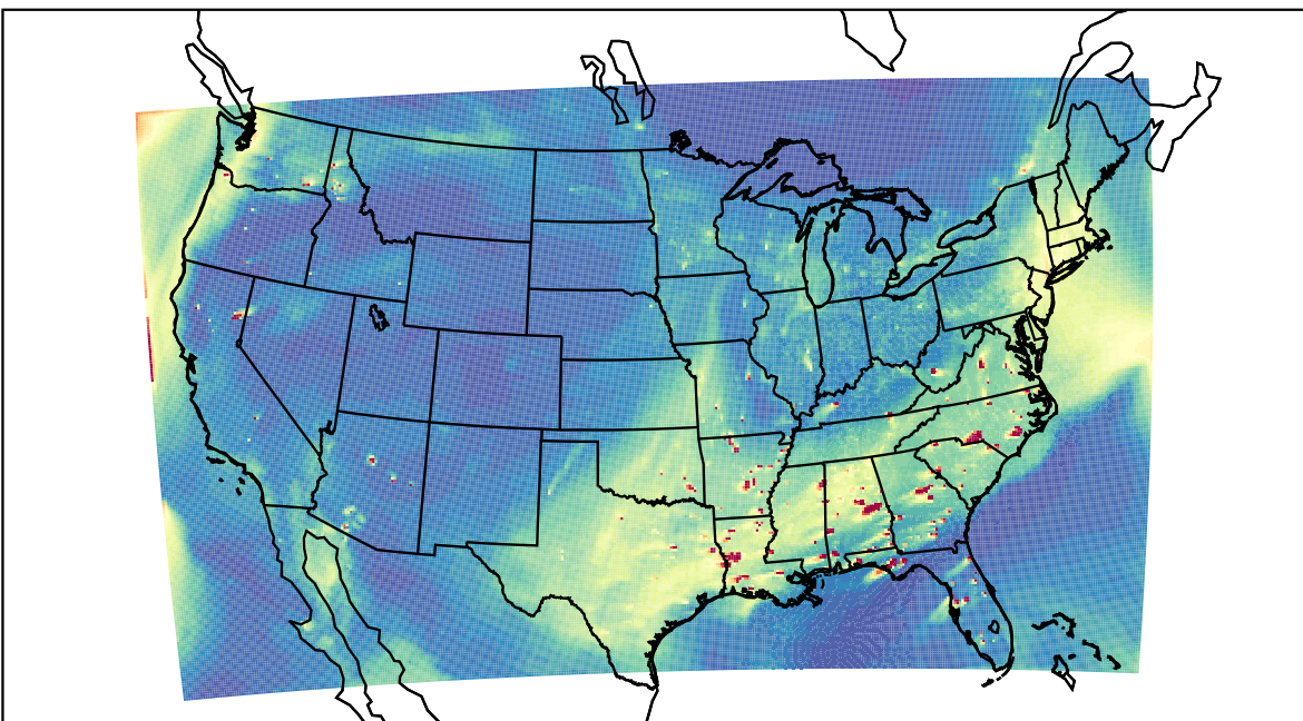
WRF 2019-09-14_23:00:00
