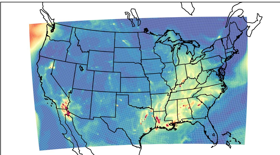
WRF 2019-09-13_14:00:00
