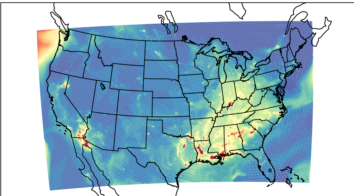
WRF 2019-09-13_12:00:00
