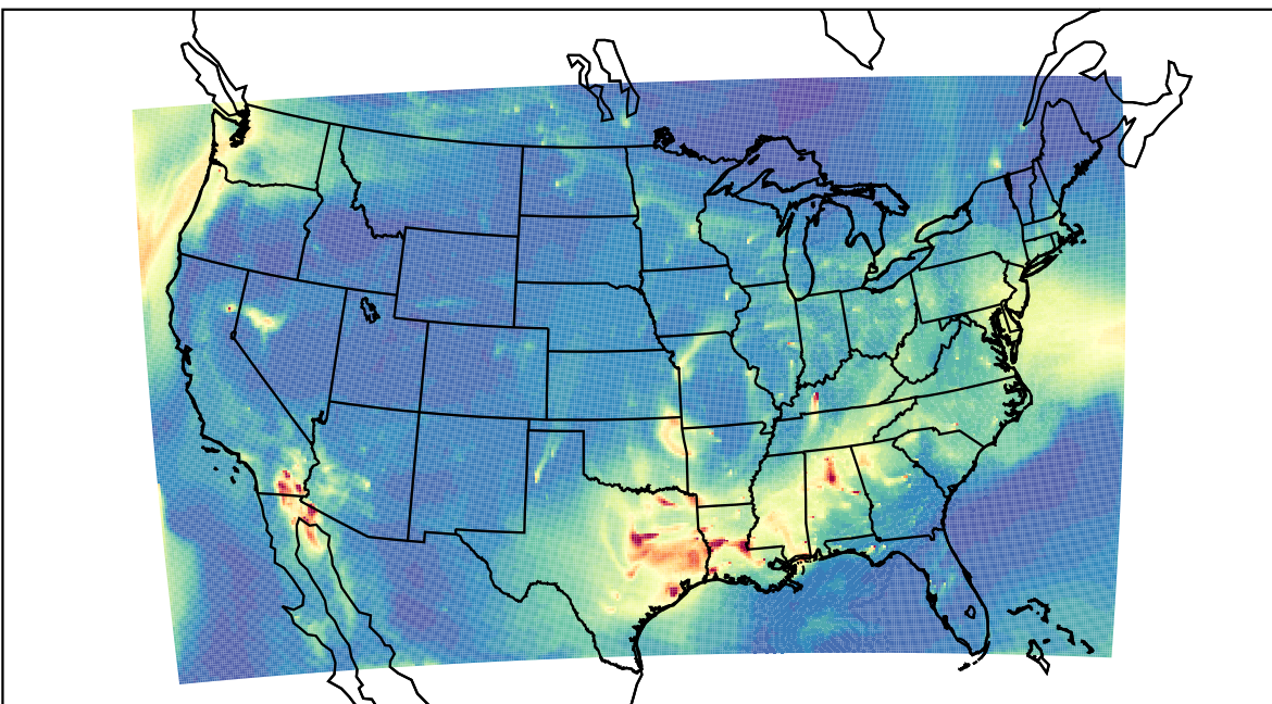
WRF 2019-09-14_12:00:00
