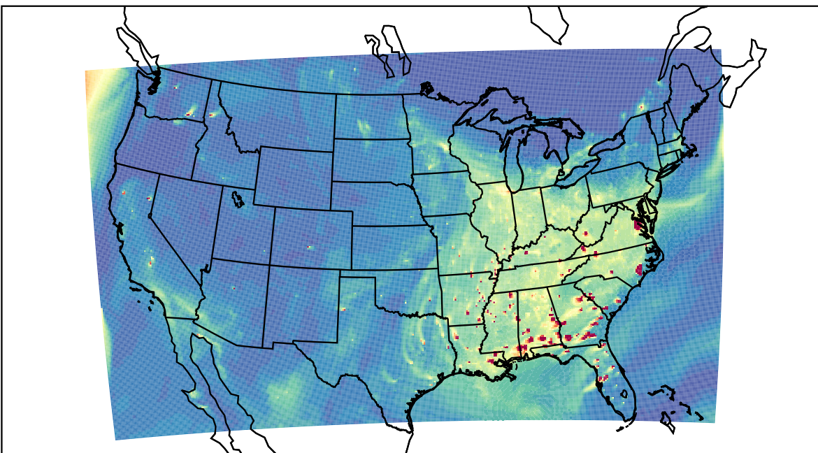
WRF 2019-09-13_00:00:00
