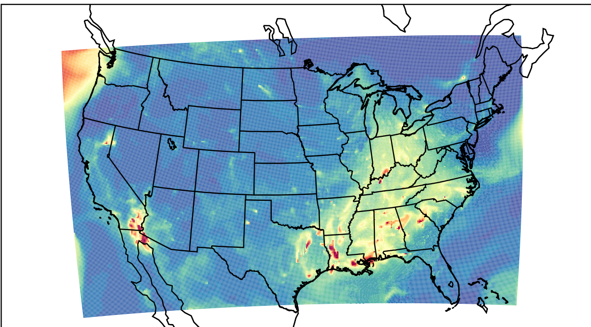
WRF 2019-09-13_13:00:00
