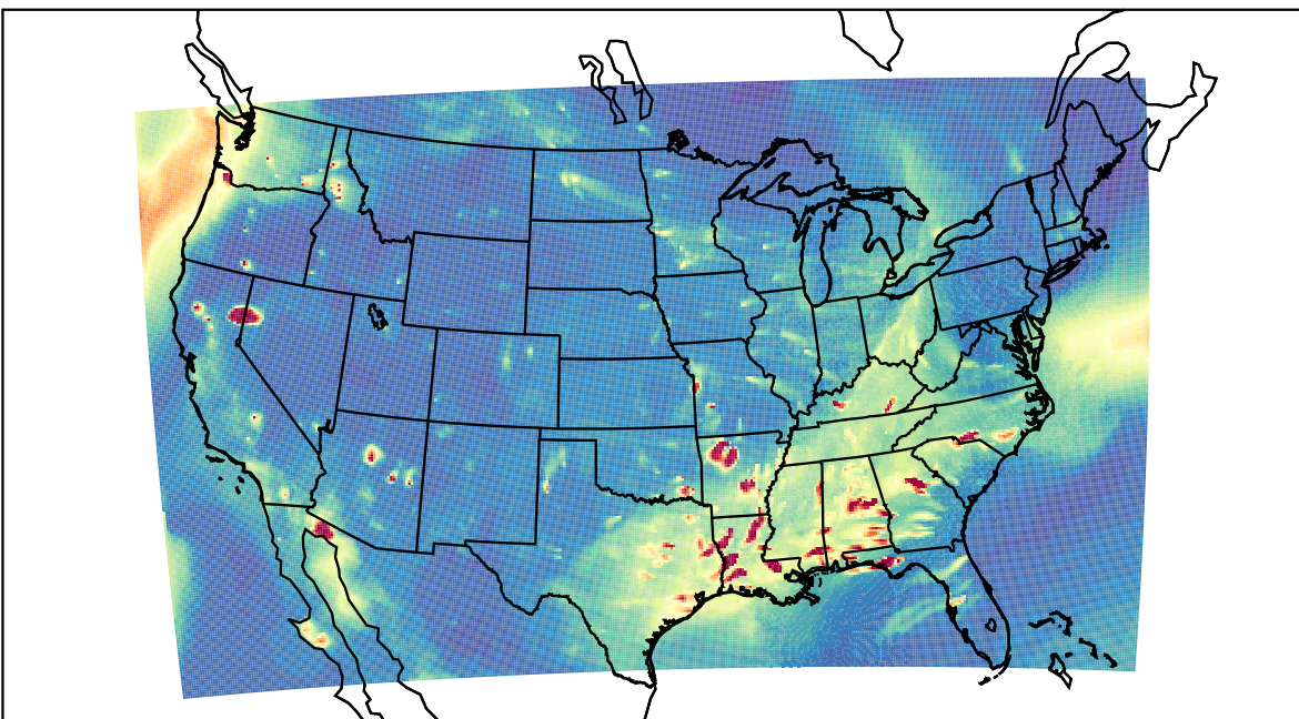
WRF 2019-09-14_03:00:00
