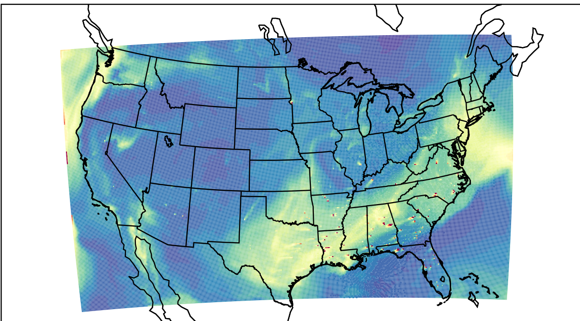
WRF 2019-09-14_19:00:00
