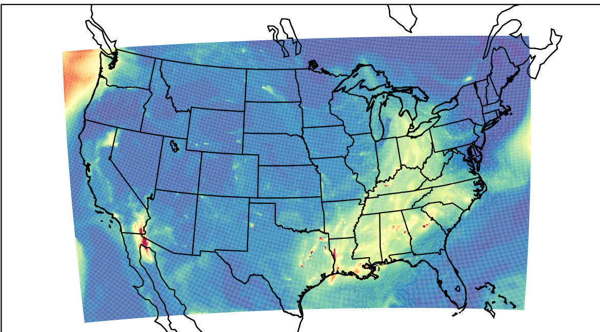
WRF 2019-09-13_16:00:00
