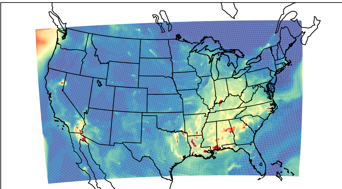
WRF 2019-09-13_10:00:00
