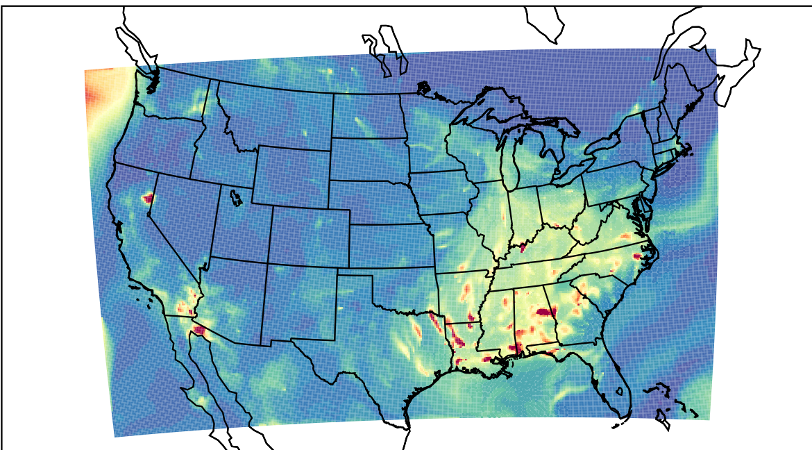
WRF 2019-09-13_07:00:00
