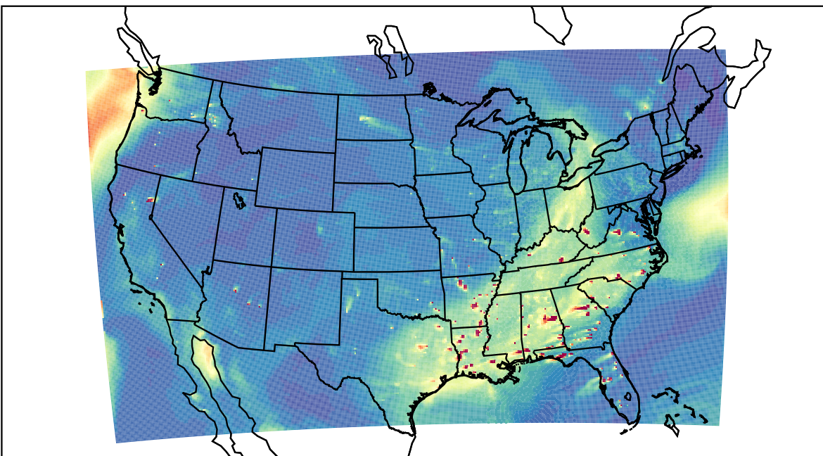
WRF 2019-09-13_23:00:00
