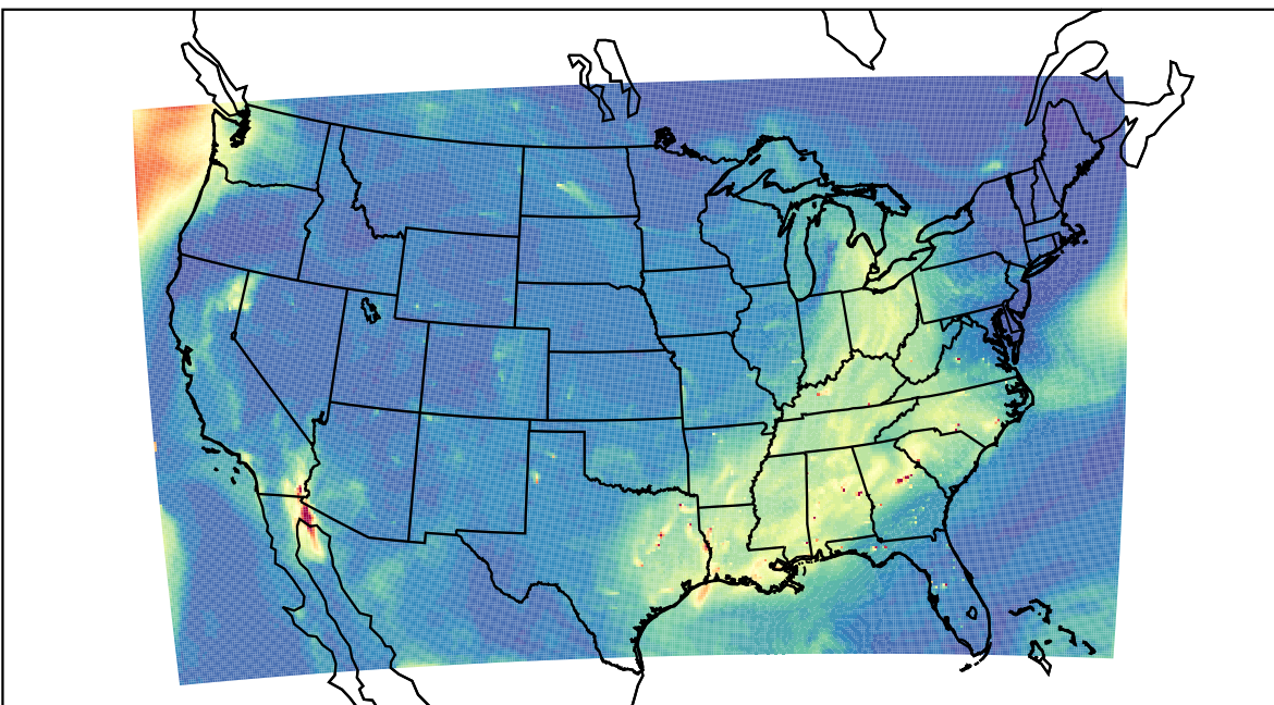
WRF 2019-09-13_17:00:00
