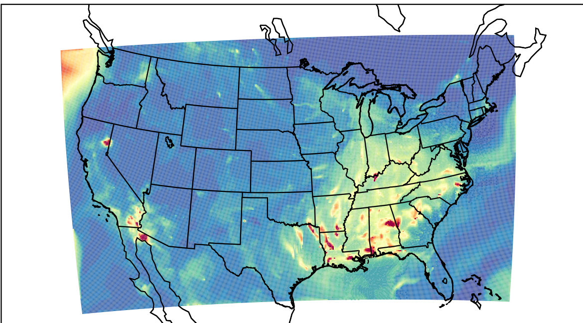
WRF 2019-09-13_08:00:00
