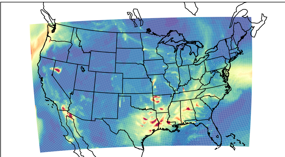
WRF 2019-09-14_07:00:00
