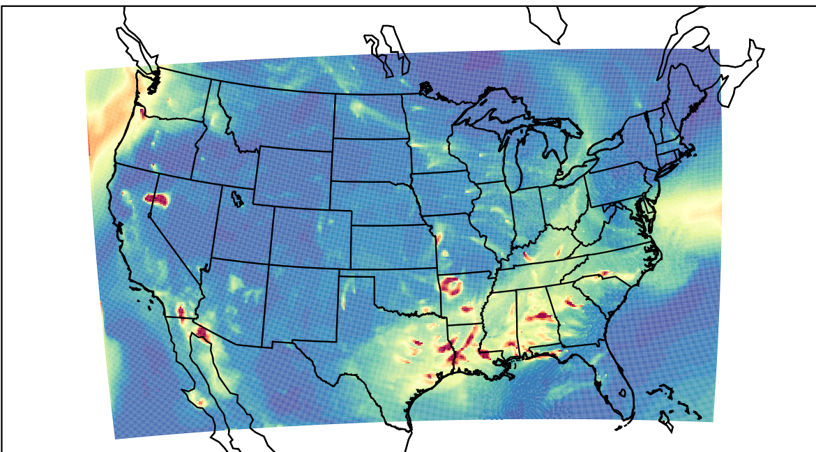
WRF 2019-09-14_05:00:00
