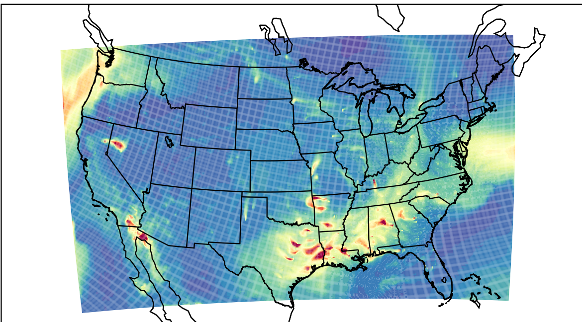
WRF 2019-09-14_08:00:00
