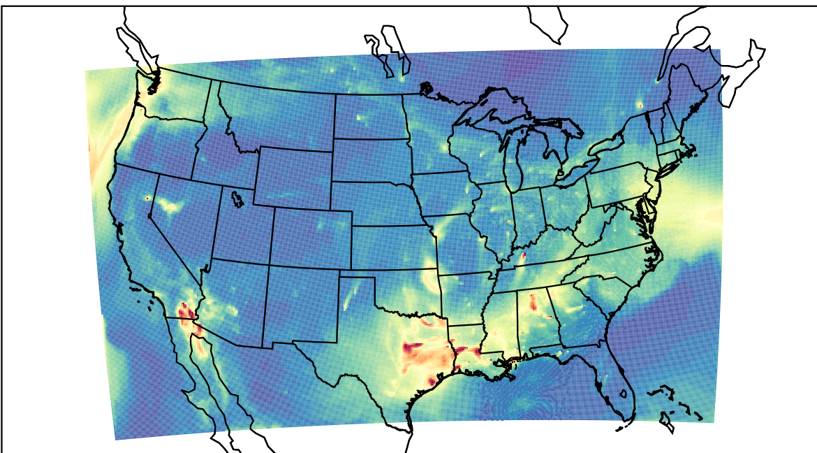
WRF 2019-09-14_13:00:00
