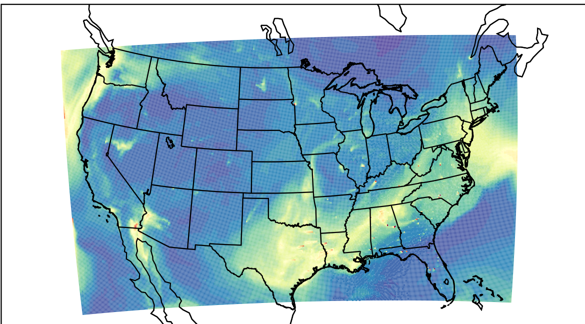
WRF 2019-09-14_17:00:00
