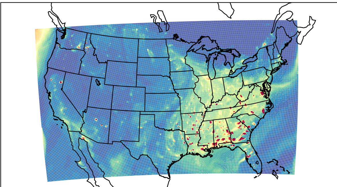
WRF 2019-09-13_01:00:00
