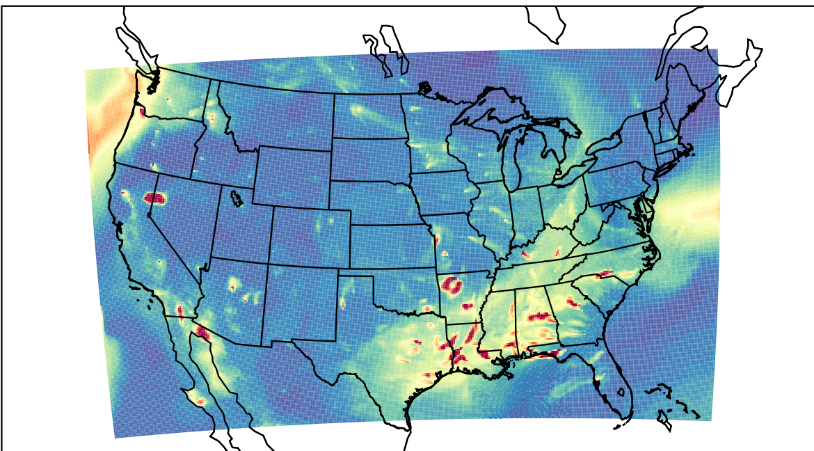
WRF 2019-09-14_04:00:00
