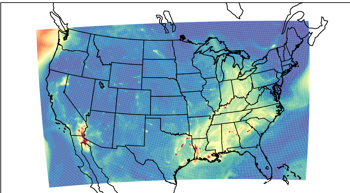
WRF 2019-09-13_15:00:00
