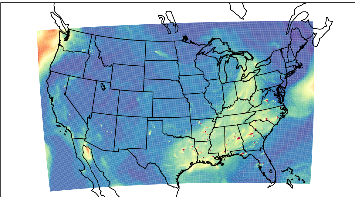
WRF 2019-09-13_20:00:00
