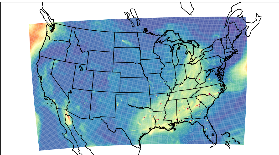
WRF 2019-09-13_19:00:00
