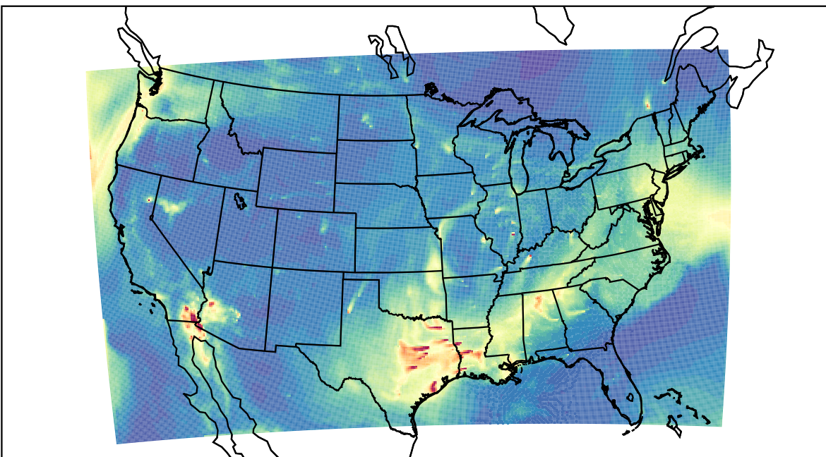
WRF 2019-09-14_15:00:00
