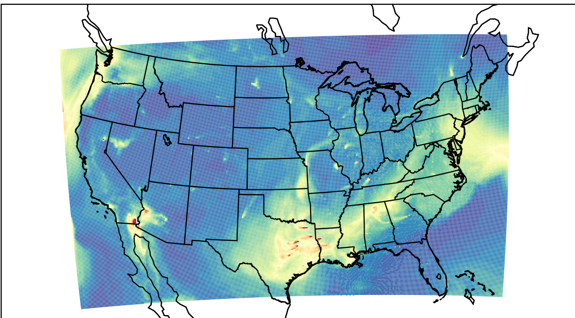
WRF 2019-09-14_16:00:00
