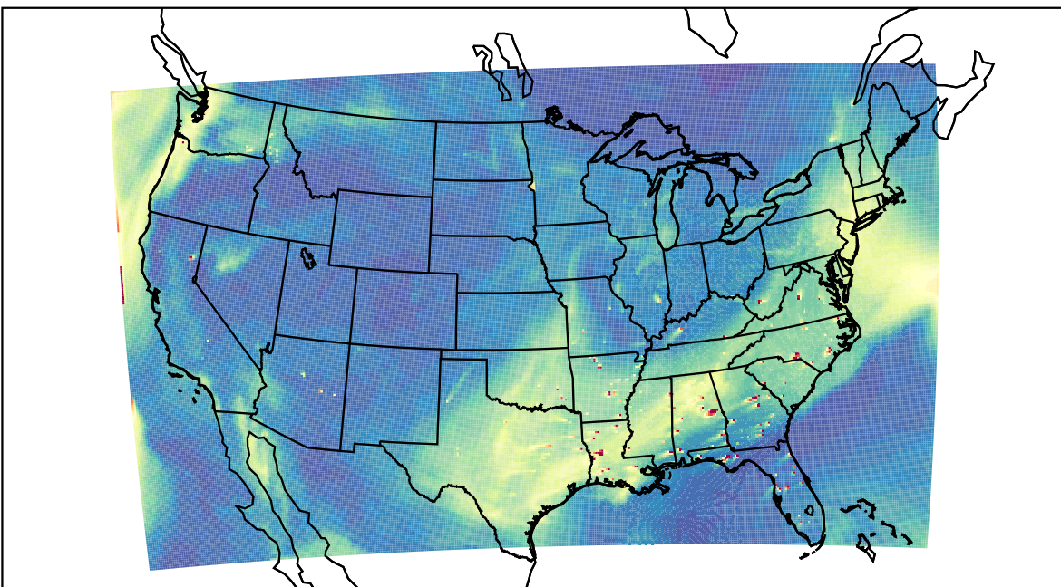
WRF 2019-09-14_20:00:00
