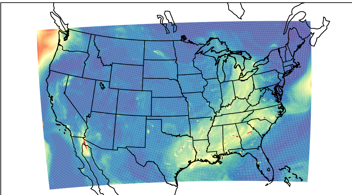
WRF 2019-09-13_18:00:00
