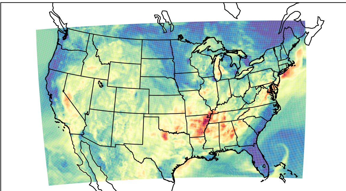
WRF (2019-09-16_04:00:00)
