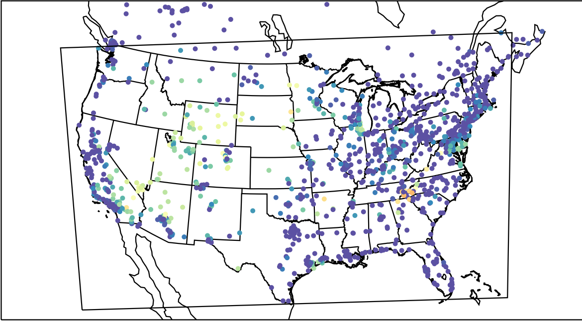
AirNOW (2019-09-17_11:00:00)
