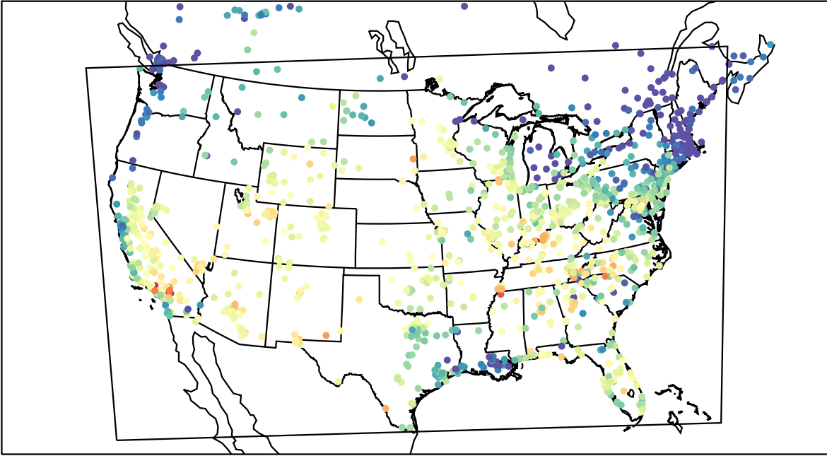
AirNOW (2019-09-17_23:00:00)
