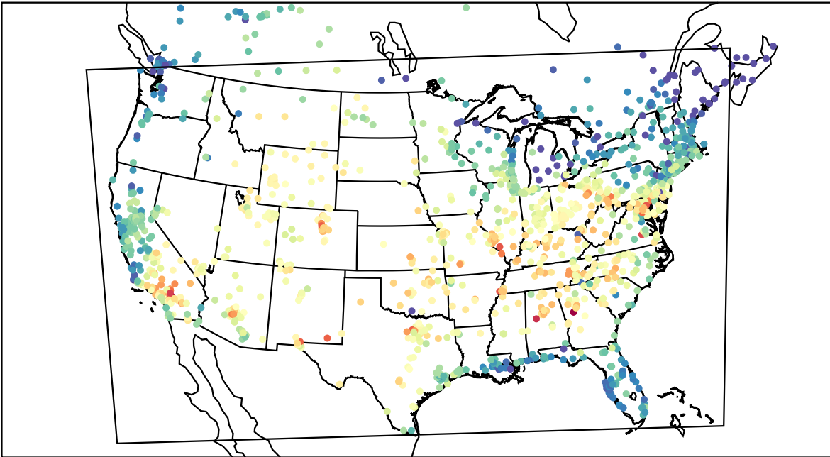
AirNOW (2019-09-16_22:00:00)
