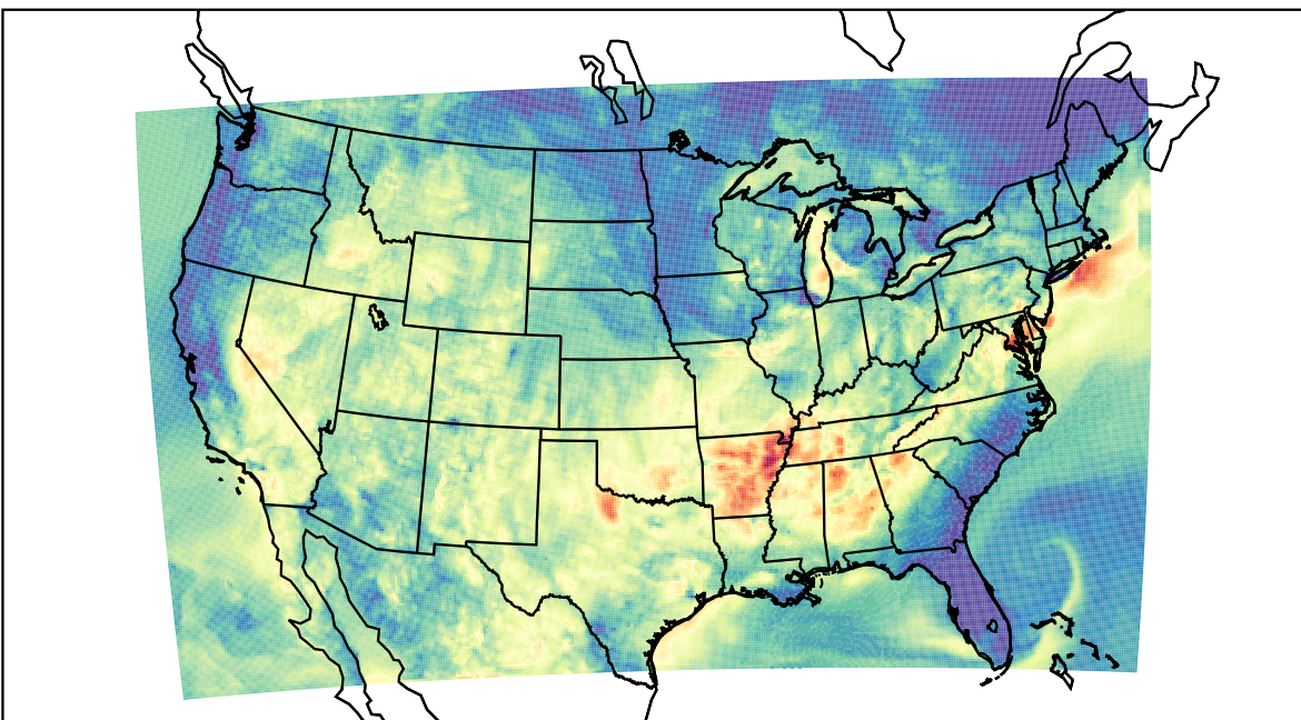
WRF (2019-09-16_06:00:00)
