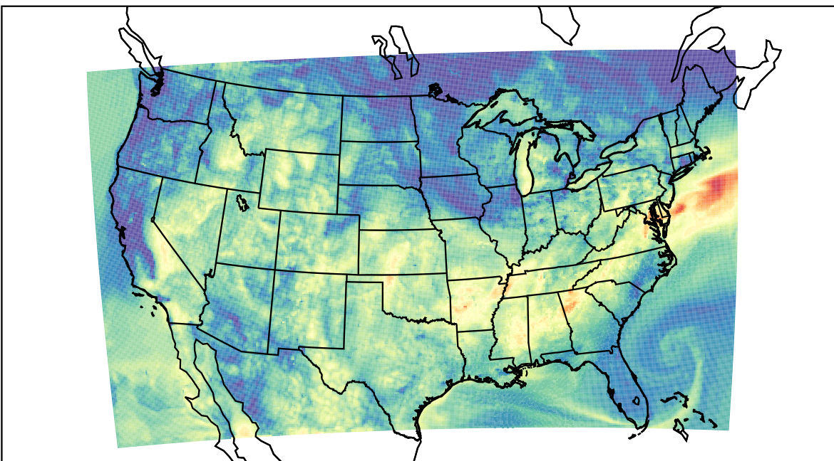
WRF (2019-09-16_14:00:00)
