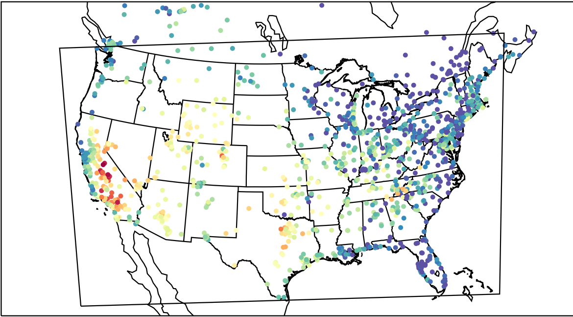
AirNOW (2019-09-16_00:00:00)
