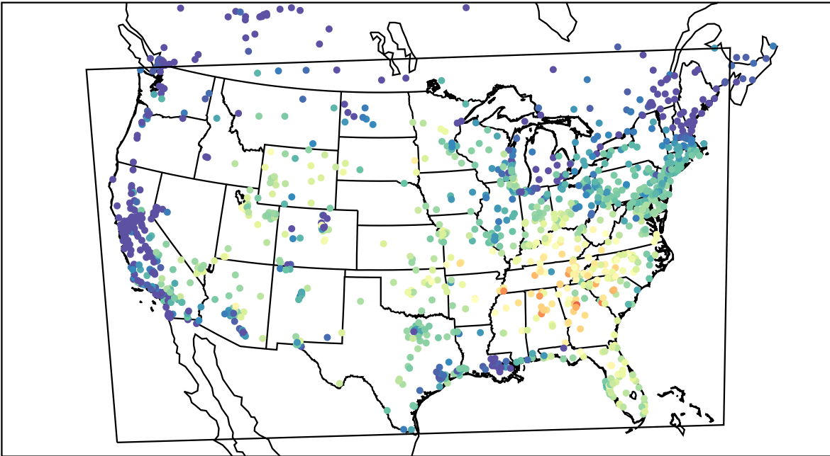
AirNOW (2019-09-17_15:00:00)
