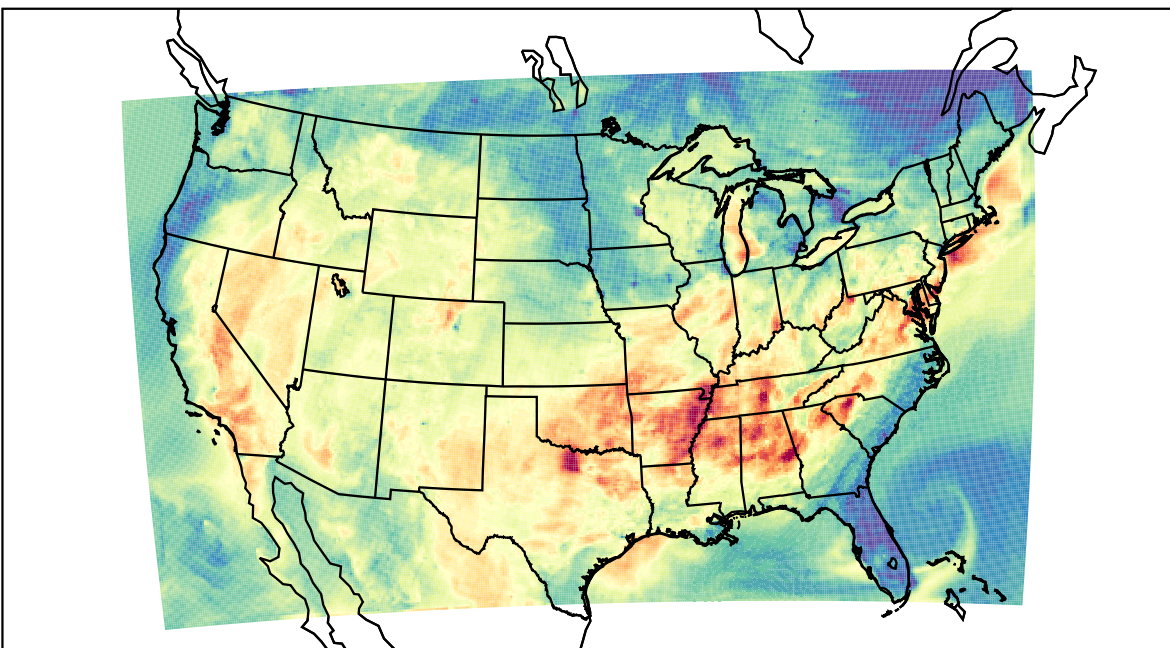
WRF (2019-09-16_01:00:00)
