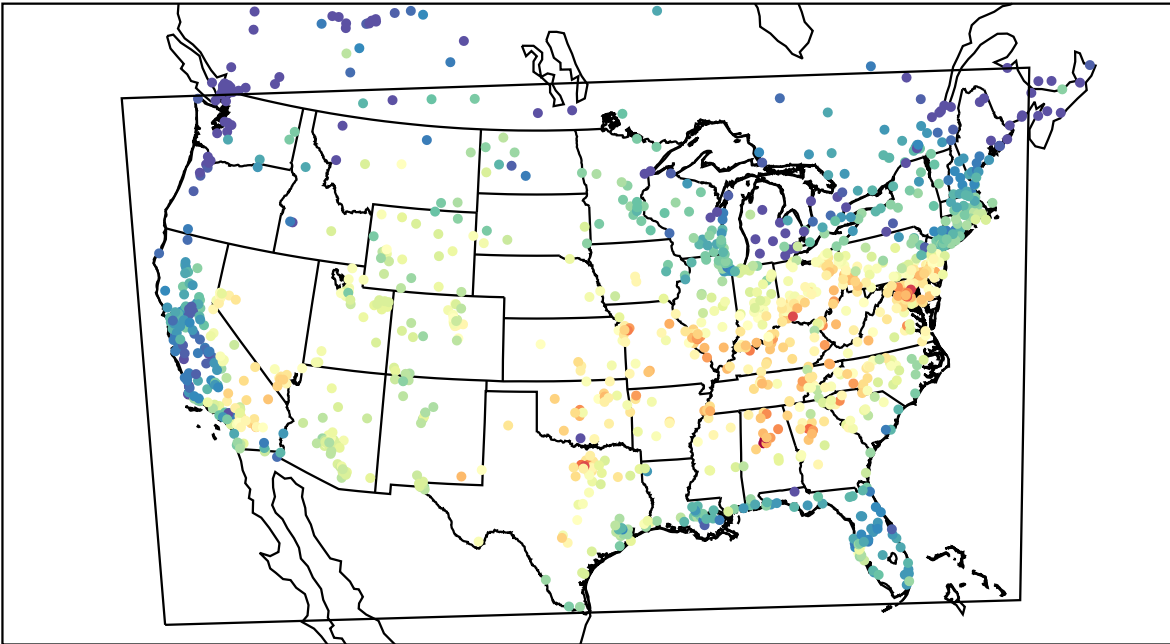
AirNOW (2019-09-16_17:00:00)
