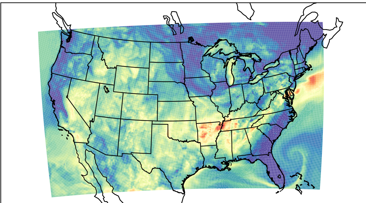
WRF (2019-09-16_11:00:00)
