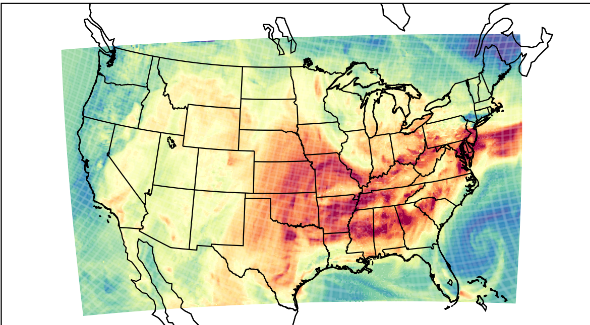
WRF (2019-09-16_20:00:00)
