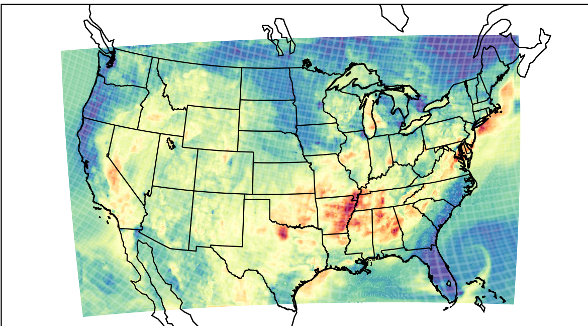
WRF (2019-09-16_03:00:00)
