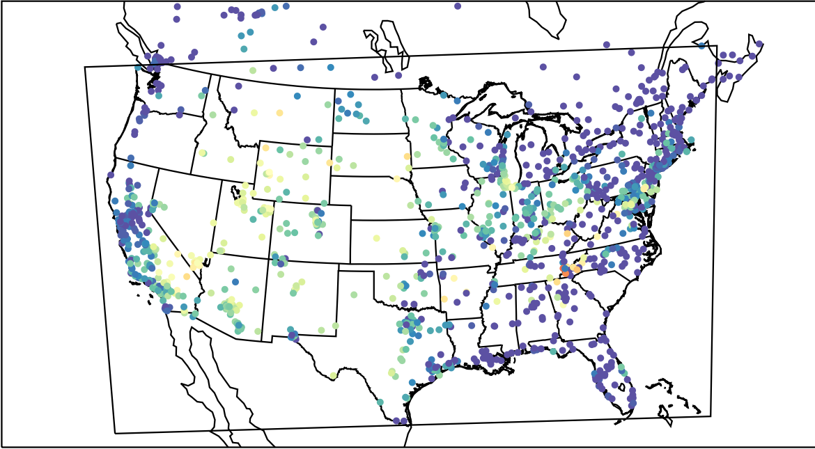
AirNOW (2019-09-17_04:00:00)
