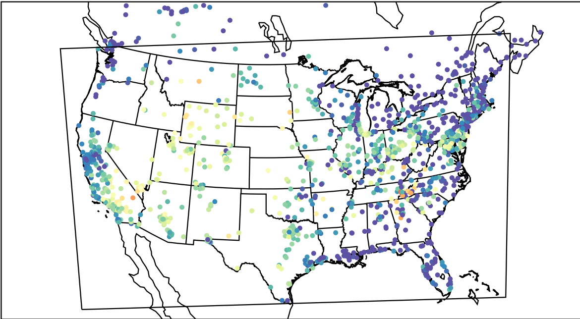
AirNOW (2019-09-17_02:00:00)
