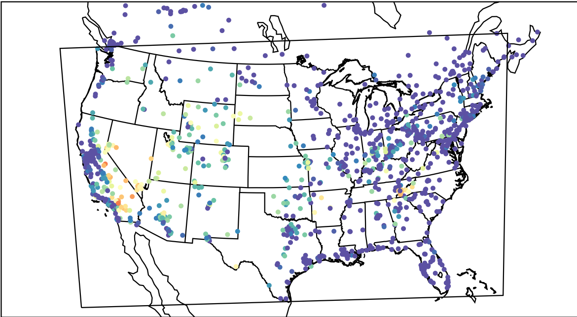
AirNOW (2019-09-16_08:00:00)
