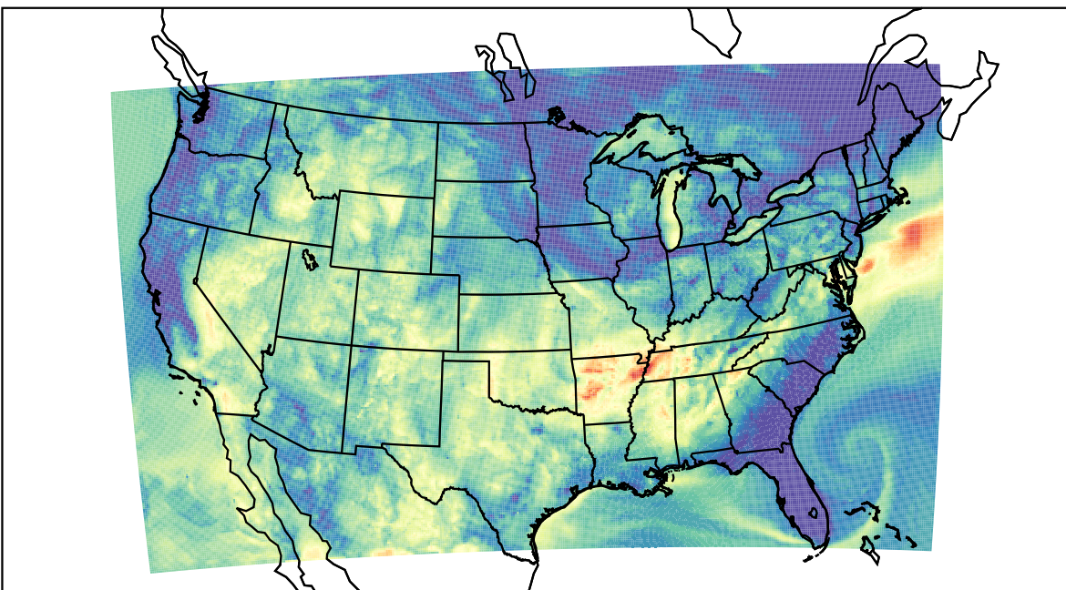
WRF (2019-09-16_12:00:00)
