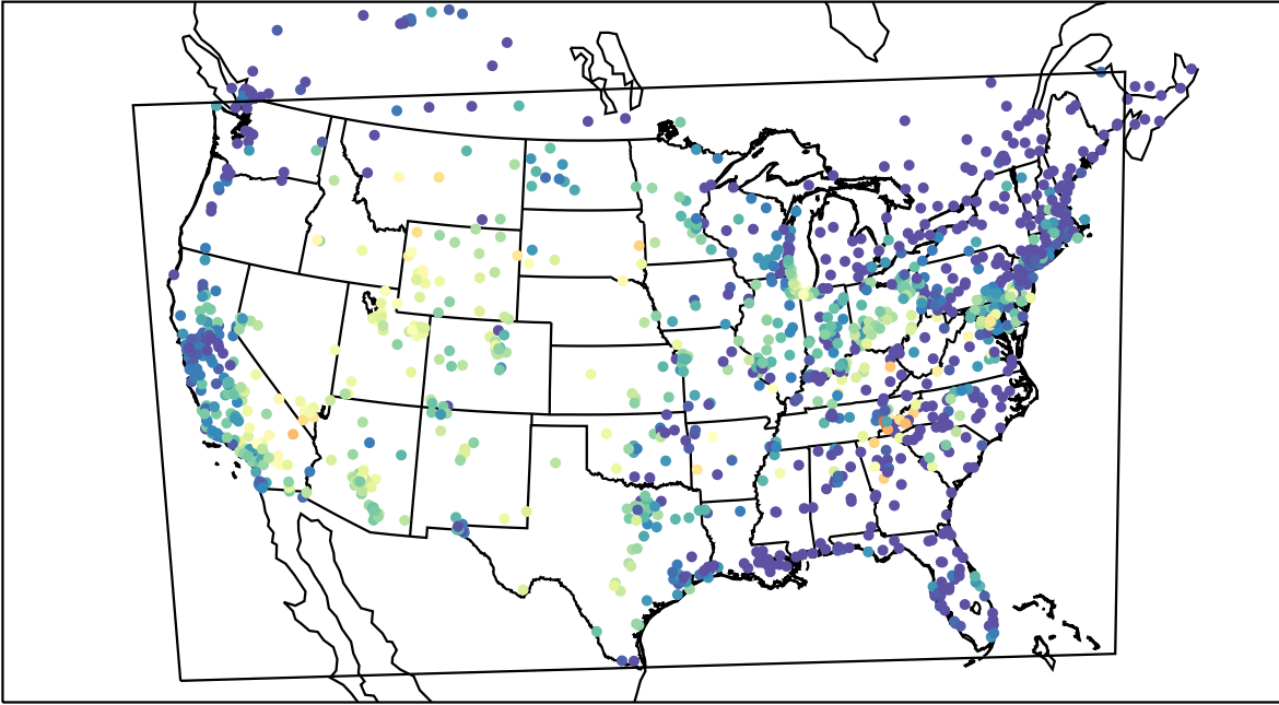
AirNOW (2019-09-17_03:00:00)
