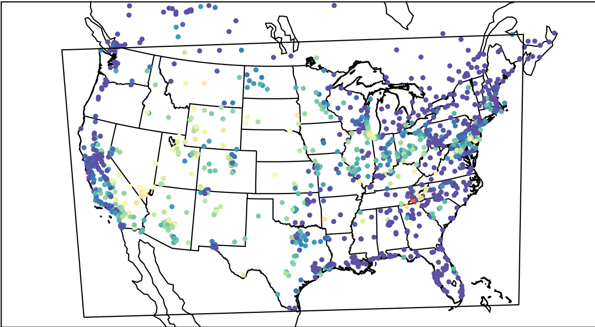
AirNOW (2019-09-17_05:00:00)
