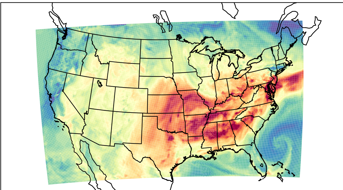
WRF (2019-09-16_18:00:00)
