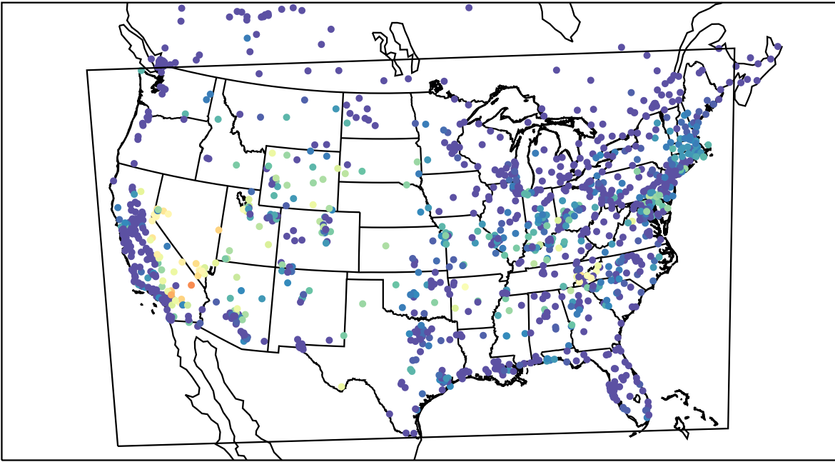
AirNOW (2019-09-16_13:00:00)
