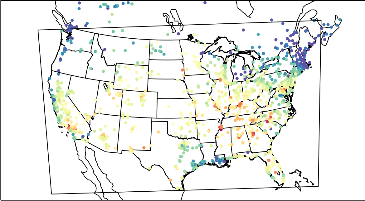
AirNOW (2019-09-17_22:00:00)
