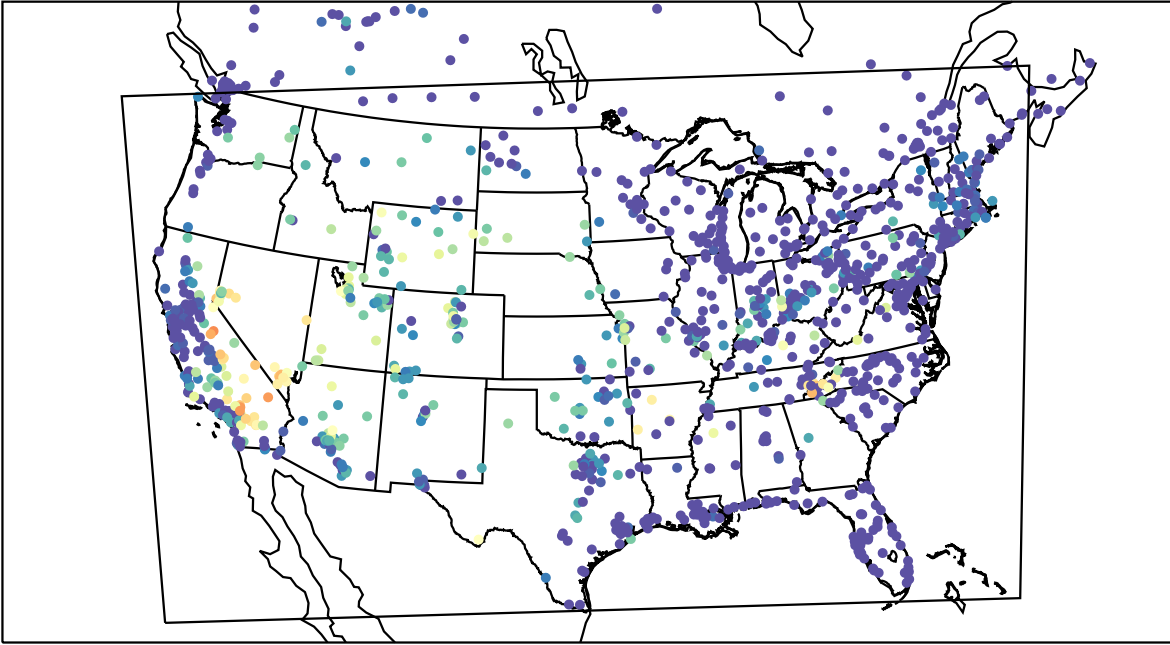
AirNOW (2019-09-16_09:00:00)
