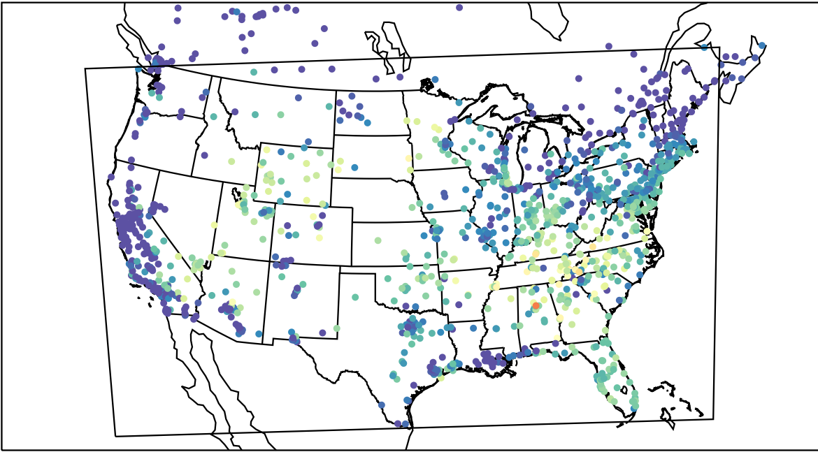
AirNOW (2019-09-17_14:00:00)
