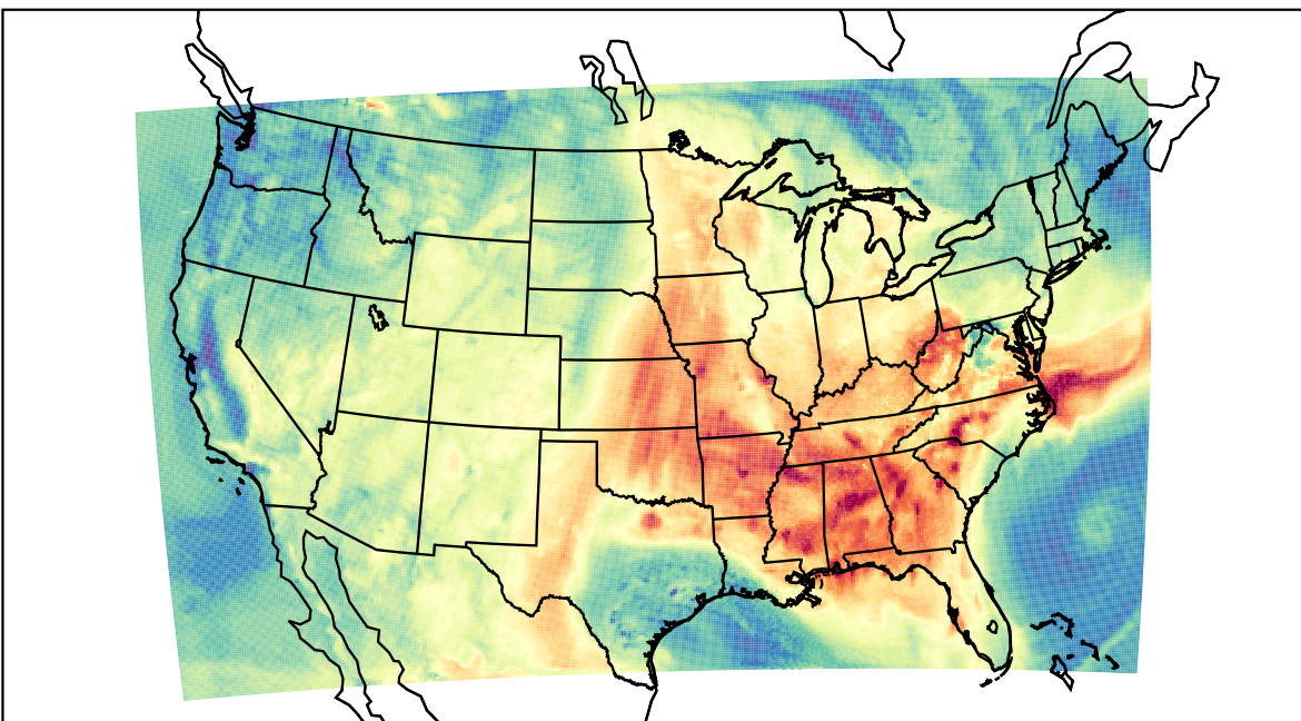
WRF (2019-09-17_17:00:00)
