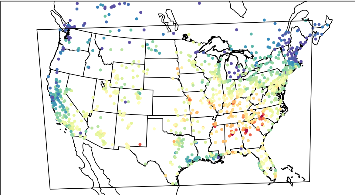
AirNOW (2019-09-17_18:00:00)
