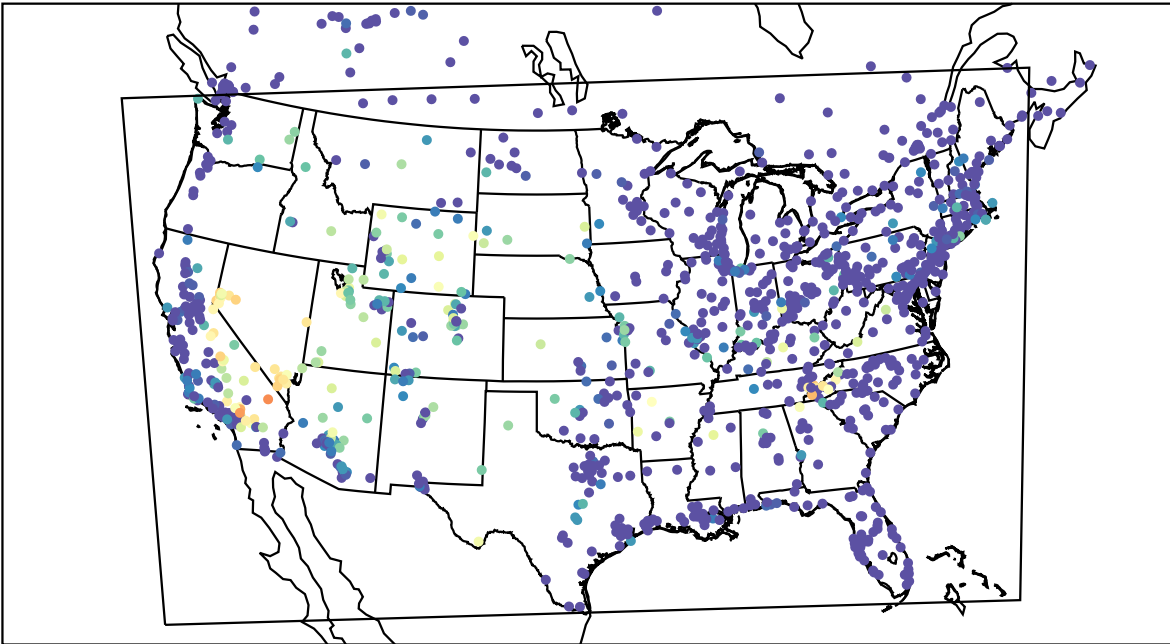
AirNOW (2019-09-16_11:00:00)
