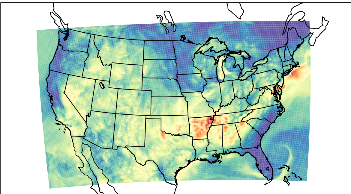
WRF (2019-09-16_07:00:00)
