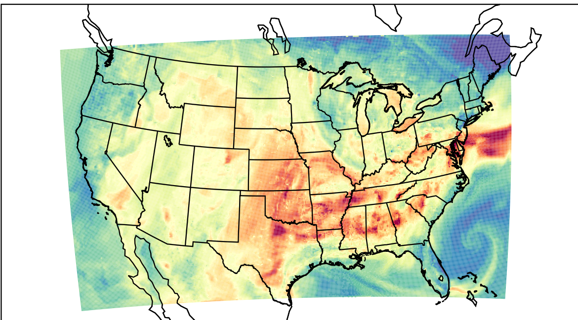
WRF (2019-09-16_23:00:00)
