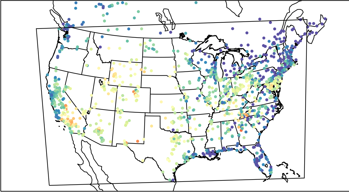
AirNOW (2019-09-17_00:00:00)
