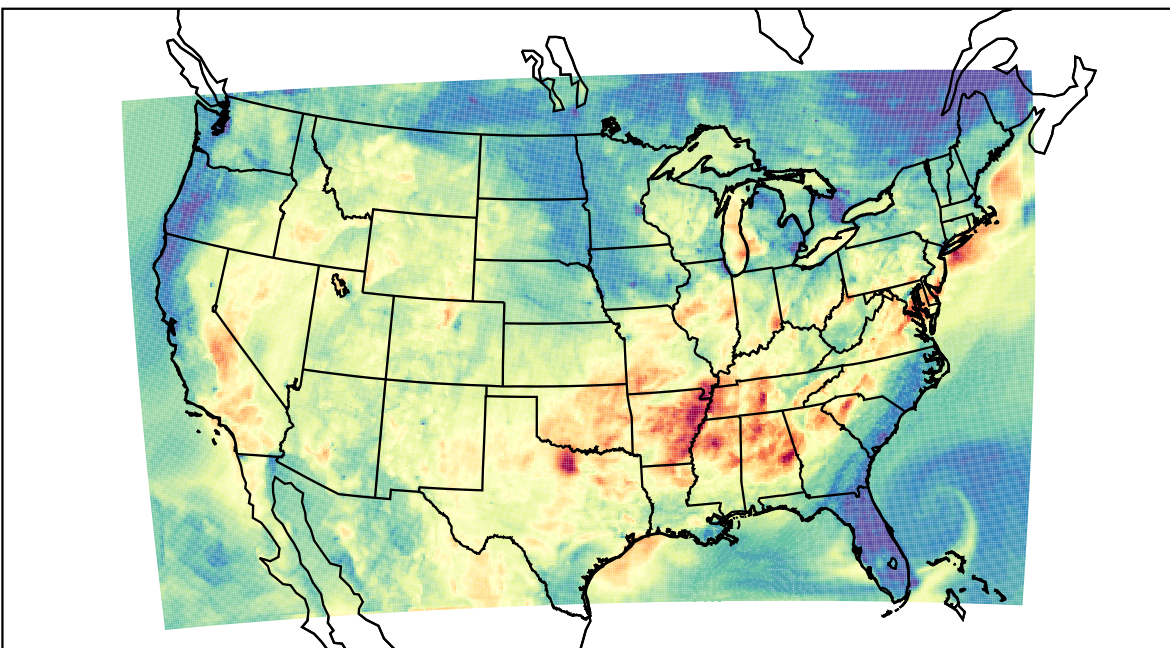
WRF (2019-09-16_02:00:00)
