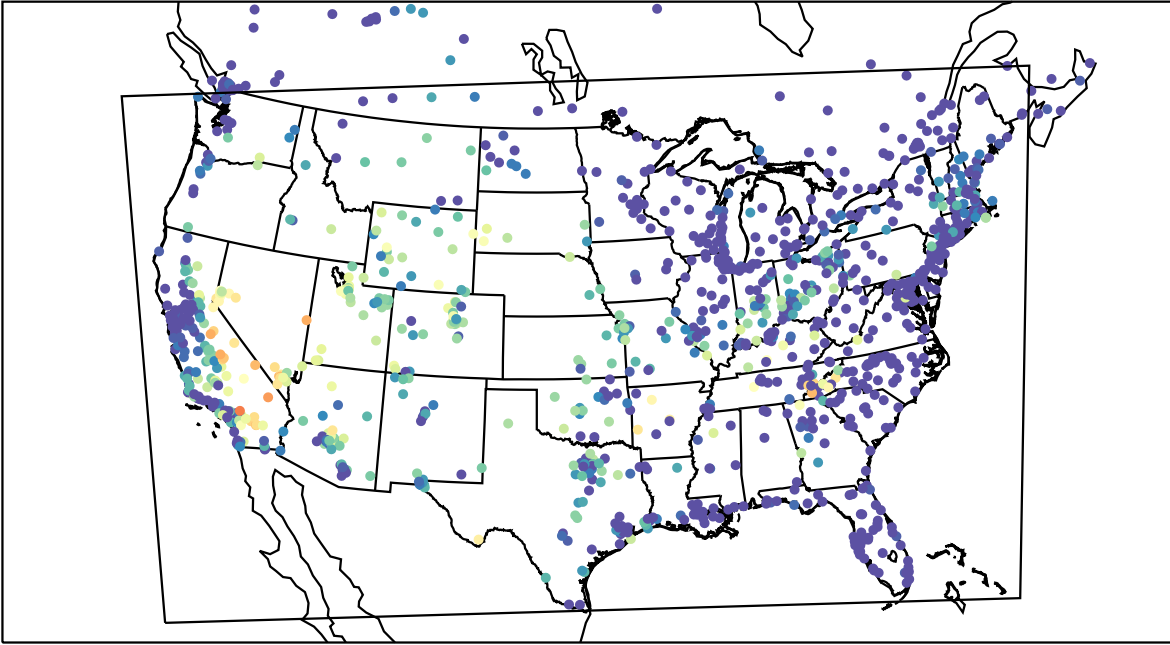
AirNOW (2019-09-16_06:00:00)
