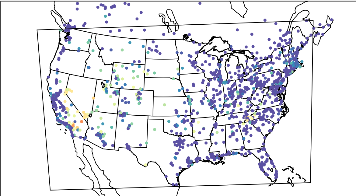
AirNOW (2019-09-16_12:00:00)
