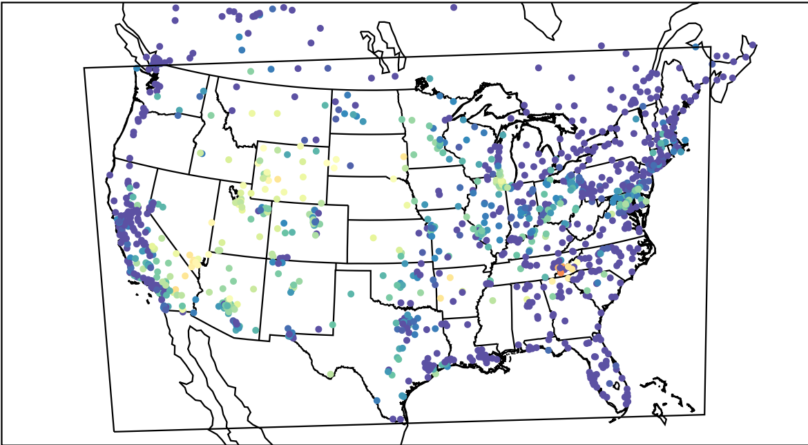
AirNOW (2019-09-17_07:00:00)
