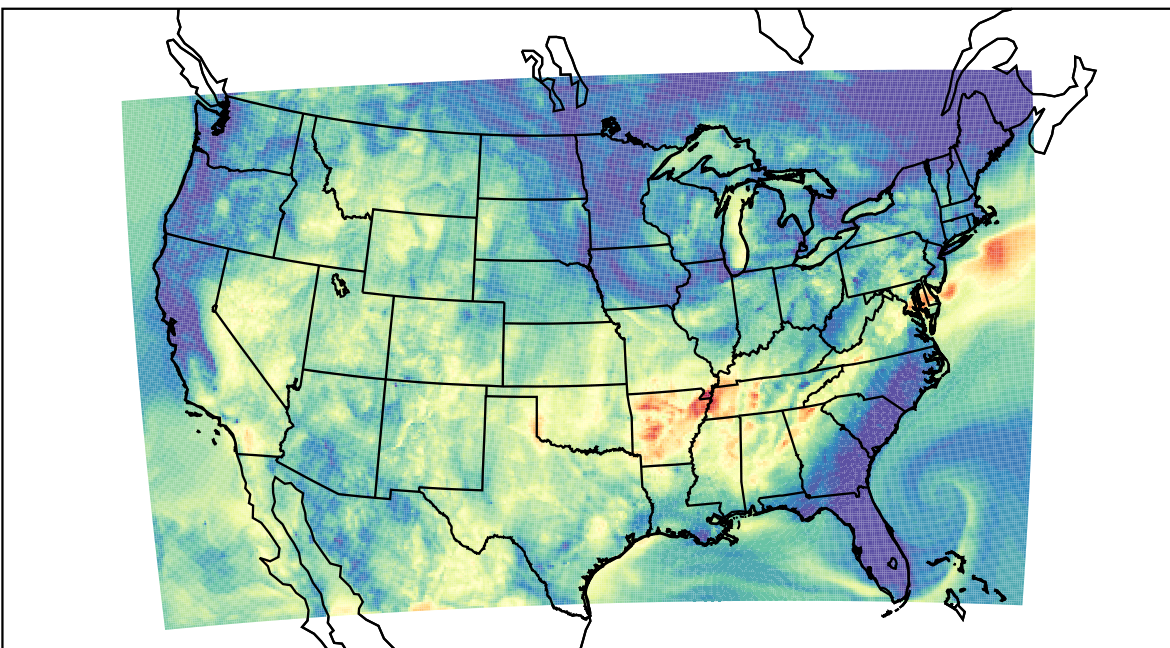
WRF (2019-09-16_10:00:00)
