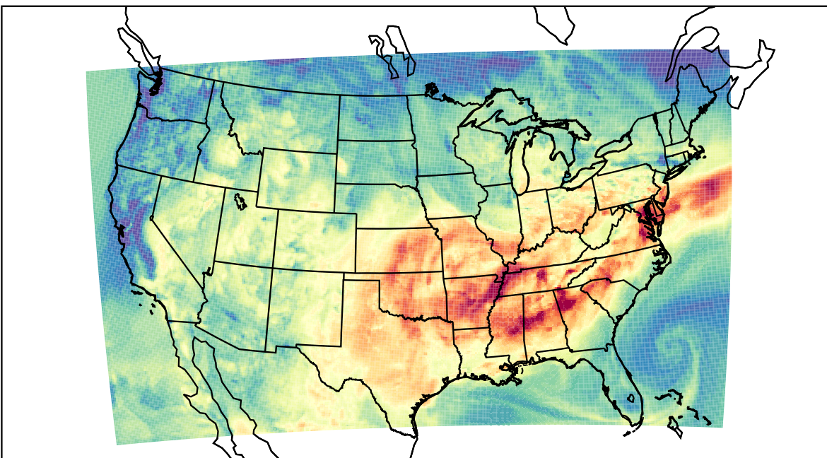
WRF (2019-09-16_16:00:00)
