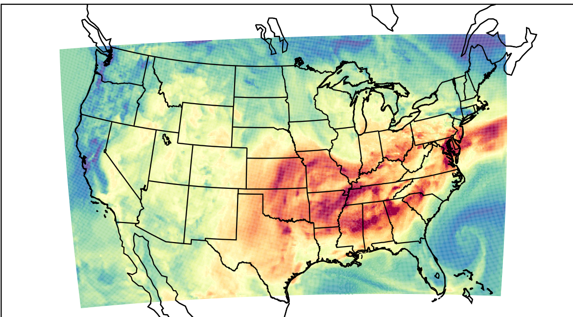
WRF (2019-09-16_17:00:00)
