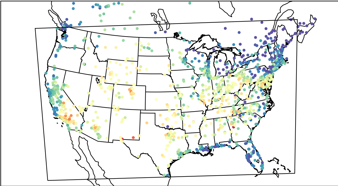
AirNOW (2019-09-16_23:00:00)
