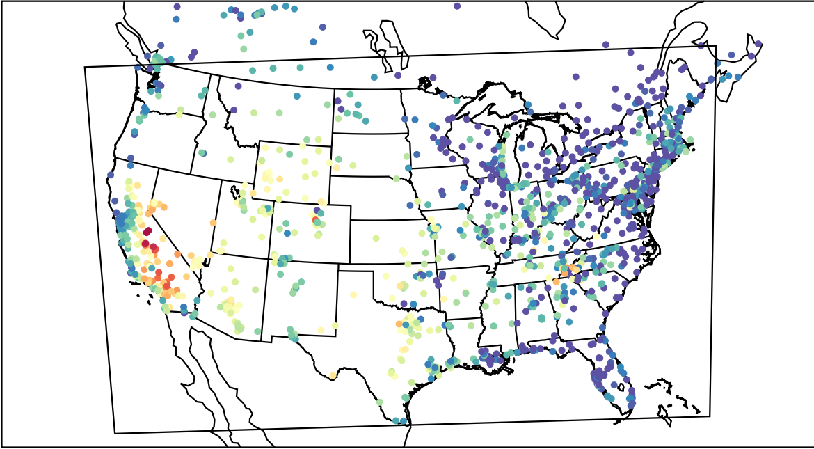
AirNOW (2019-09-16_01:00:00)
