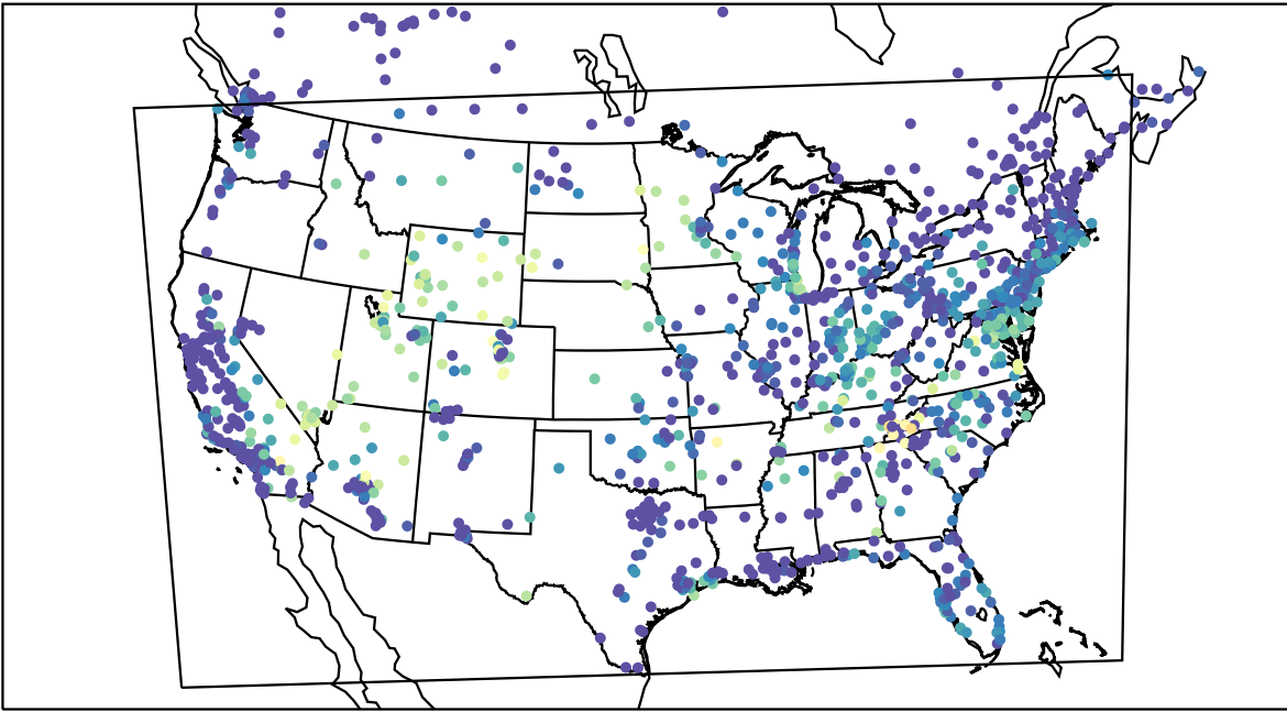
AirNOW (2019-09-17_13:00:00)
