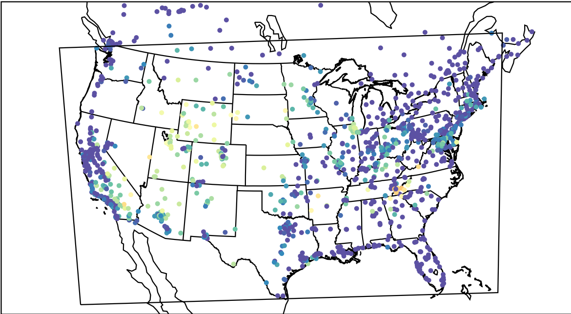
AirNOW (2019-09-17_08:00:00)
