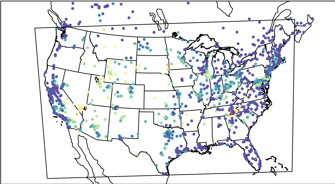
AirNOW (2019-09-17_06:00:00)
