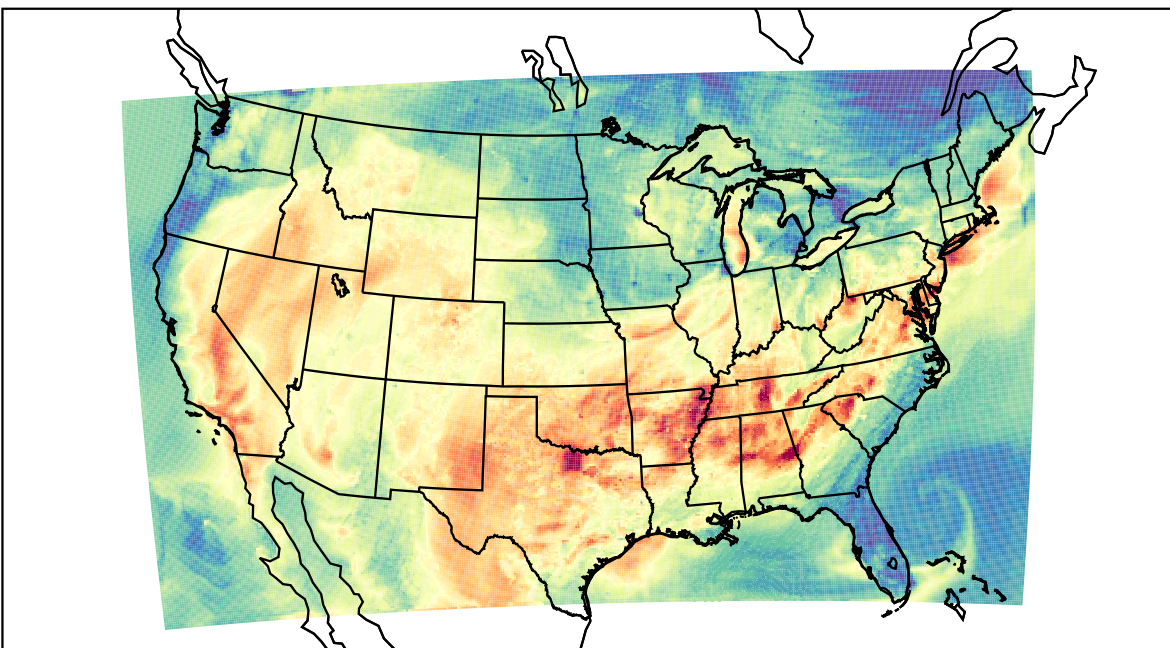
WRF (2019-09-16_00:00:00)
