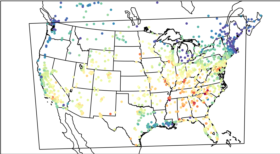
AirNOW (2019-09-17_21:00:00)
