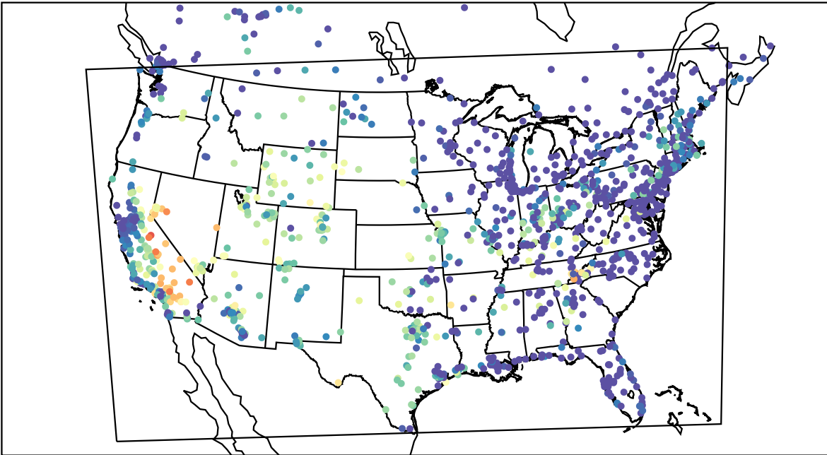
AirNOW (2019-09-16_04:00:00)
