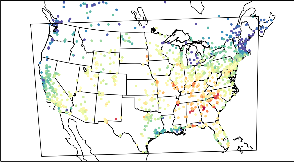
AirNOW (2019-09-17_19:00:00)
