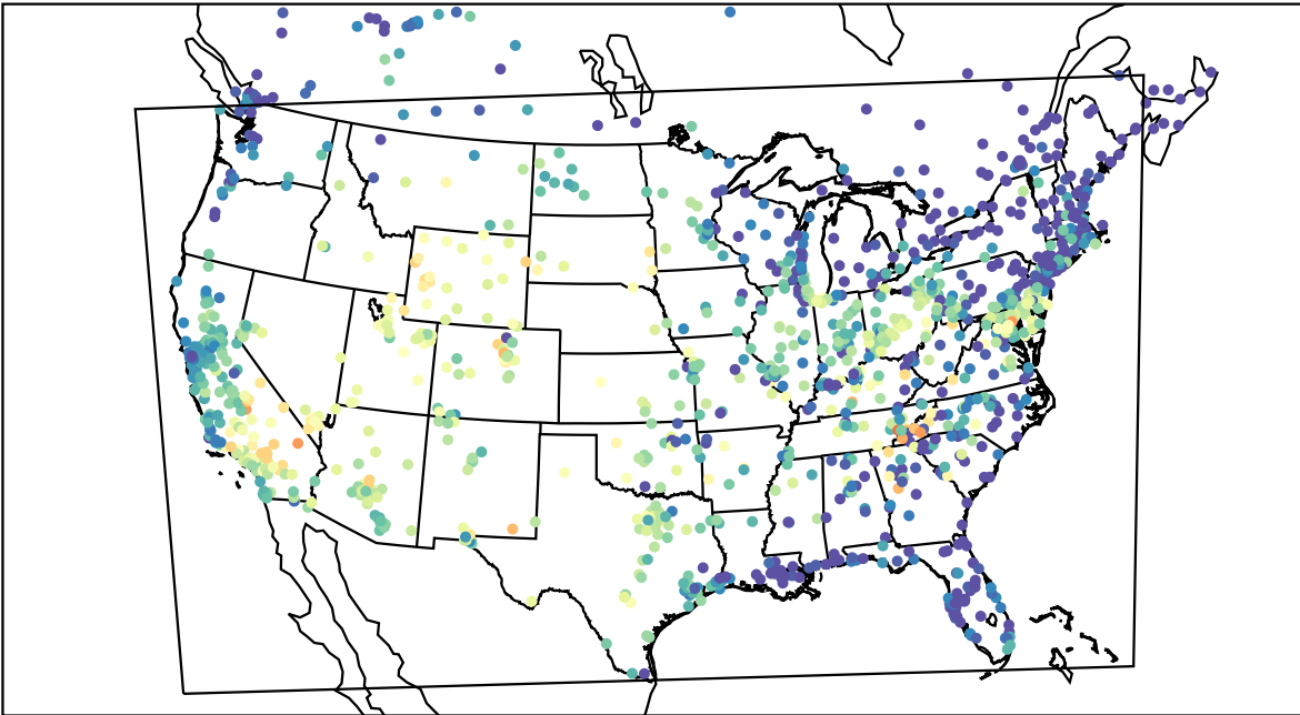
AirNOW (2019-09-17_01:00:00)
