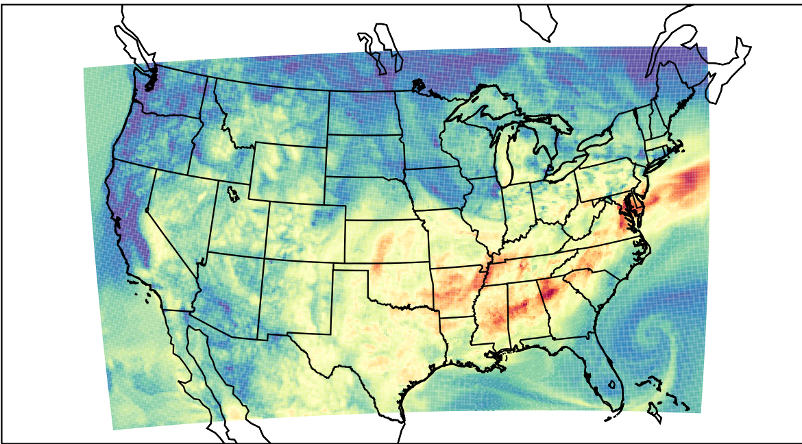
WRF (2019-09-16_15:00:00)
