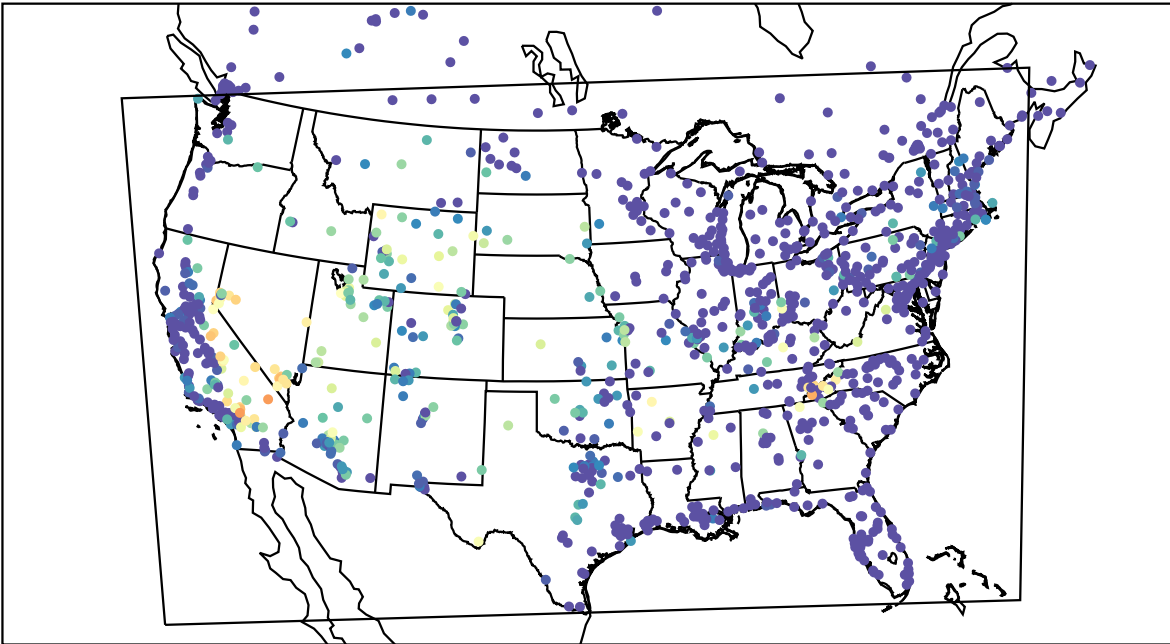
AirNOW (2019-09-16_10:00:00)
