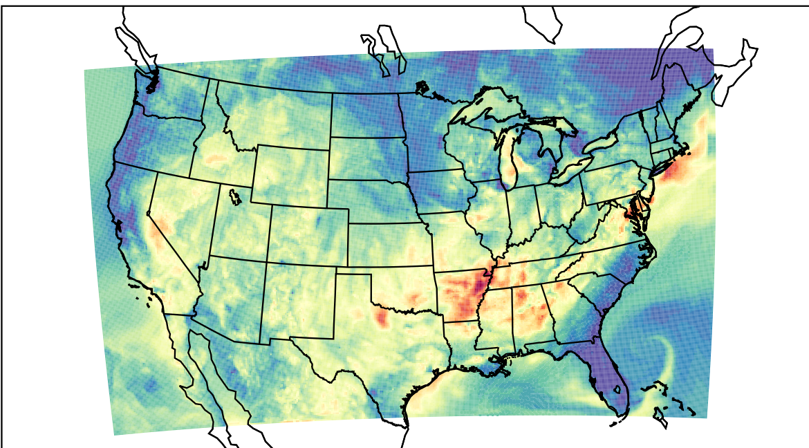
WRF (2019-09-16_05:00:00)
