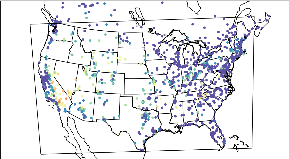
AirNOW (2019-09-16_07:00:00)
