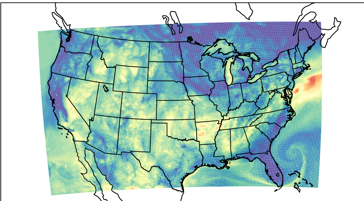
WRF (2019-09-16_13:00:00)
