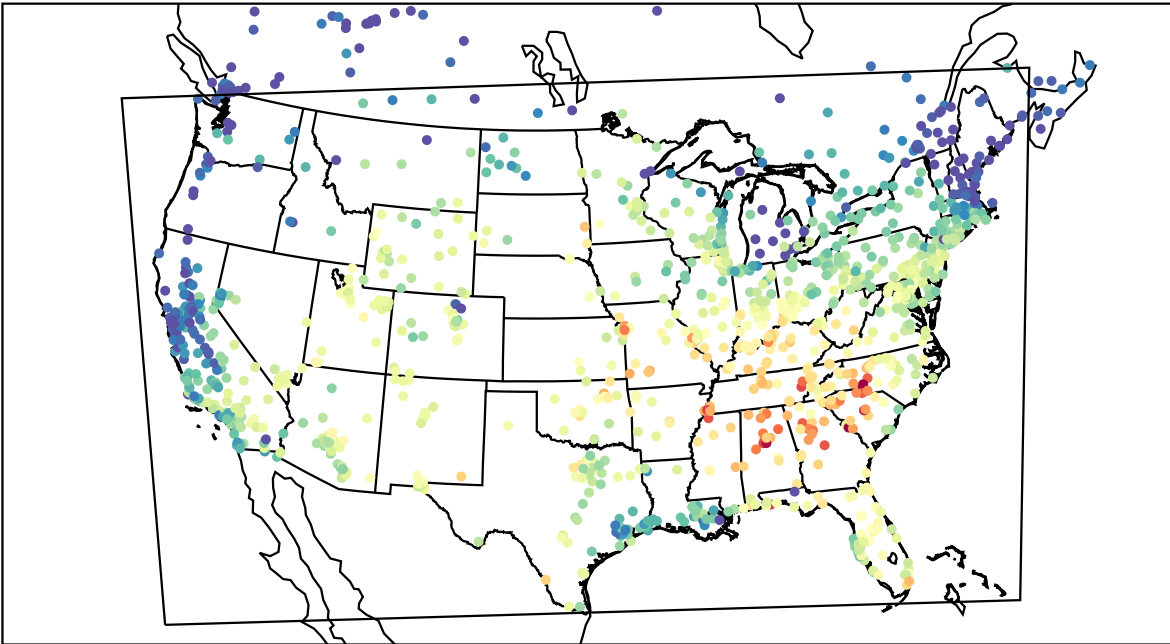
AirNOW (2019-09-17_17:00:00)
