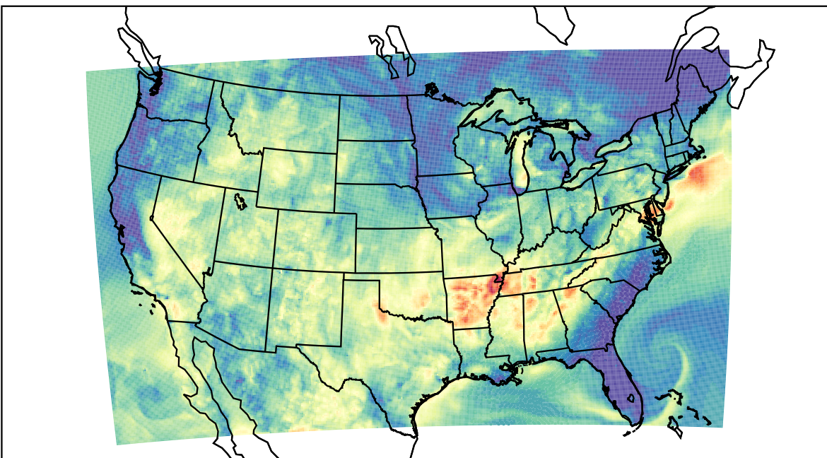
WRF (2019-09-16_08:00:00)
