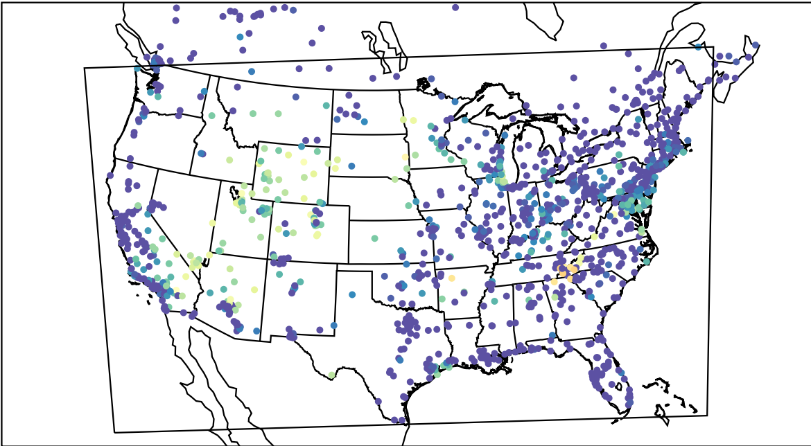
AirNOW (2019-09-17_12:00:00)
