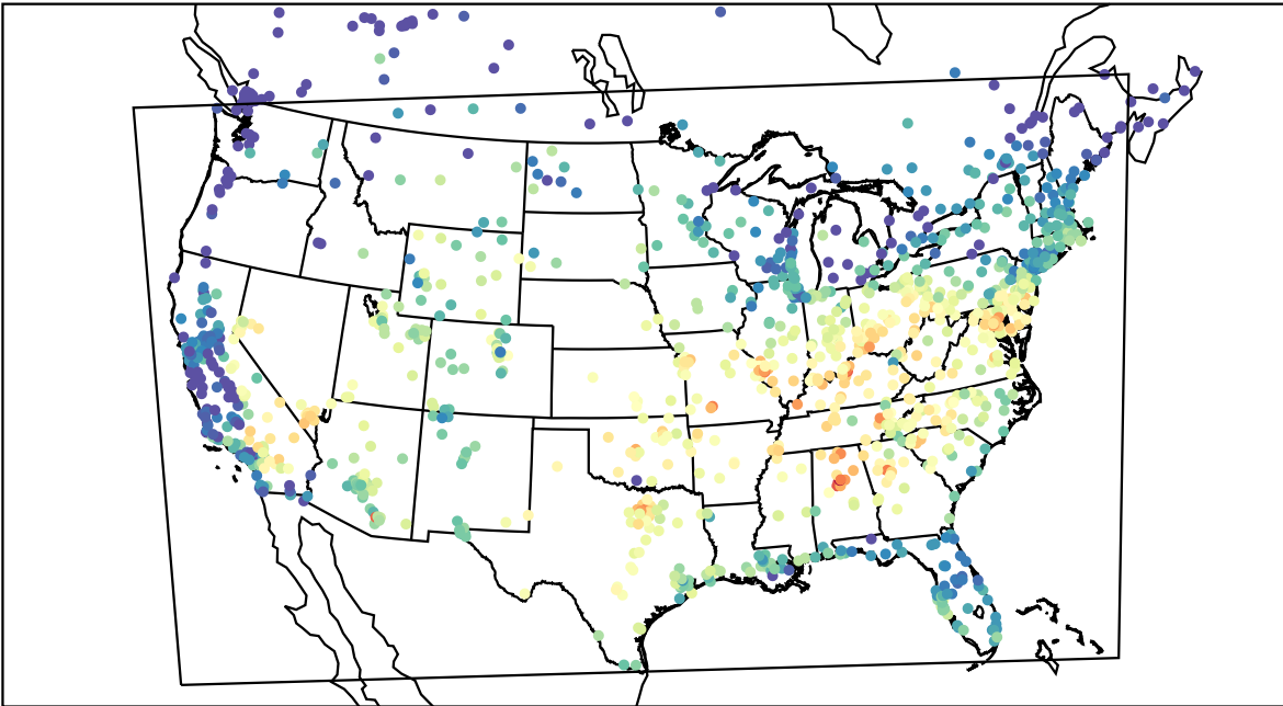
AirNOW (2019-09-16_16:00:00)
