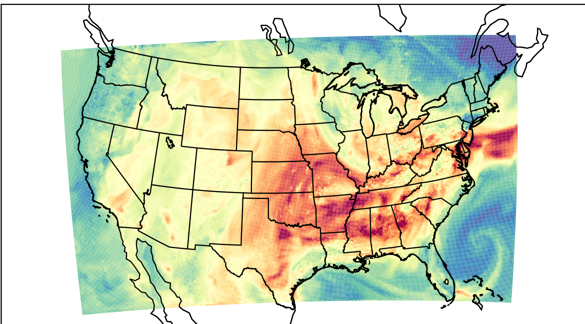
WRF (2019-09-16_22:00:00)
