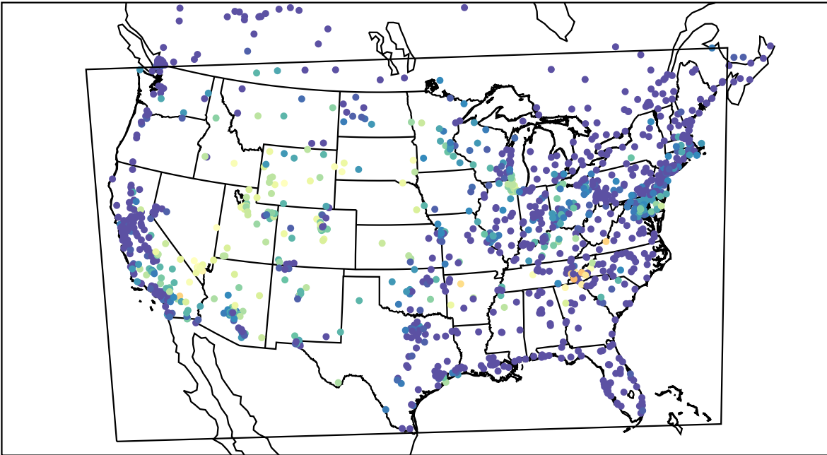
AirNOW (2019-09-17_09:00:00)
