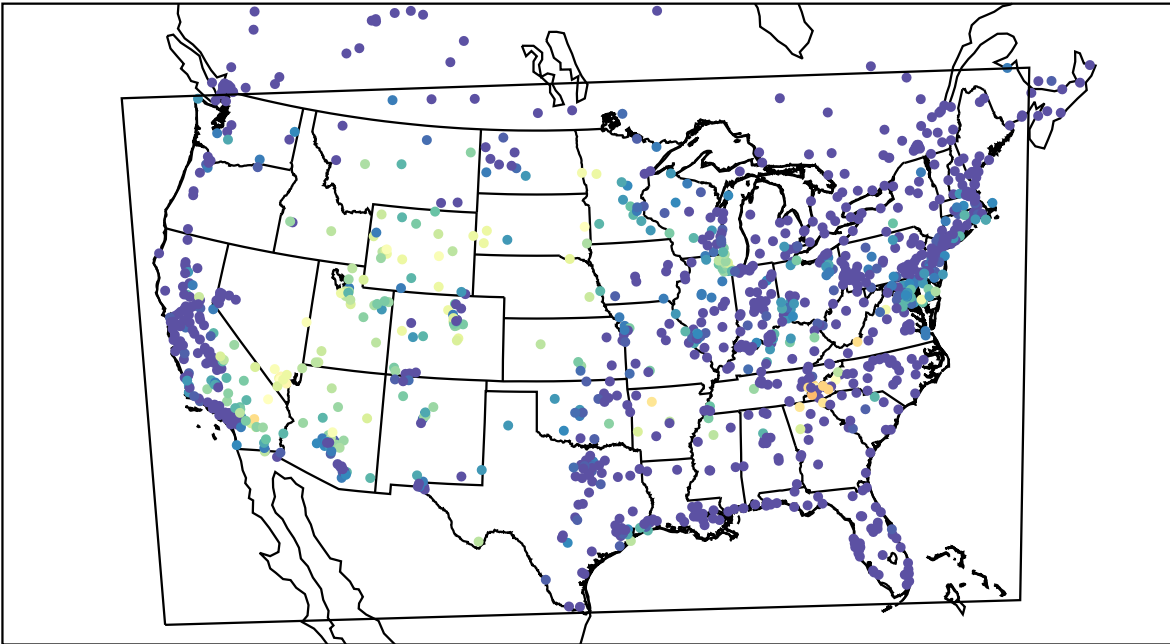
AirNOW (2019-09-17_10:00:00)
