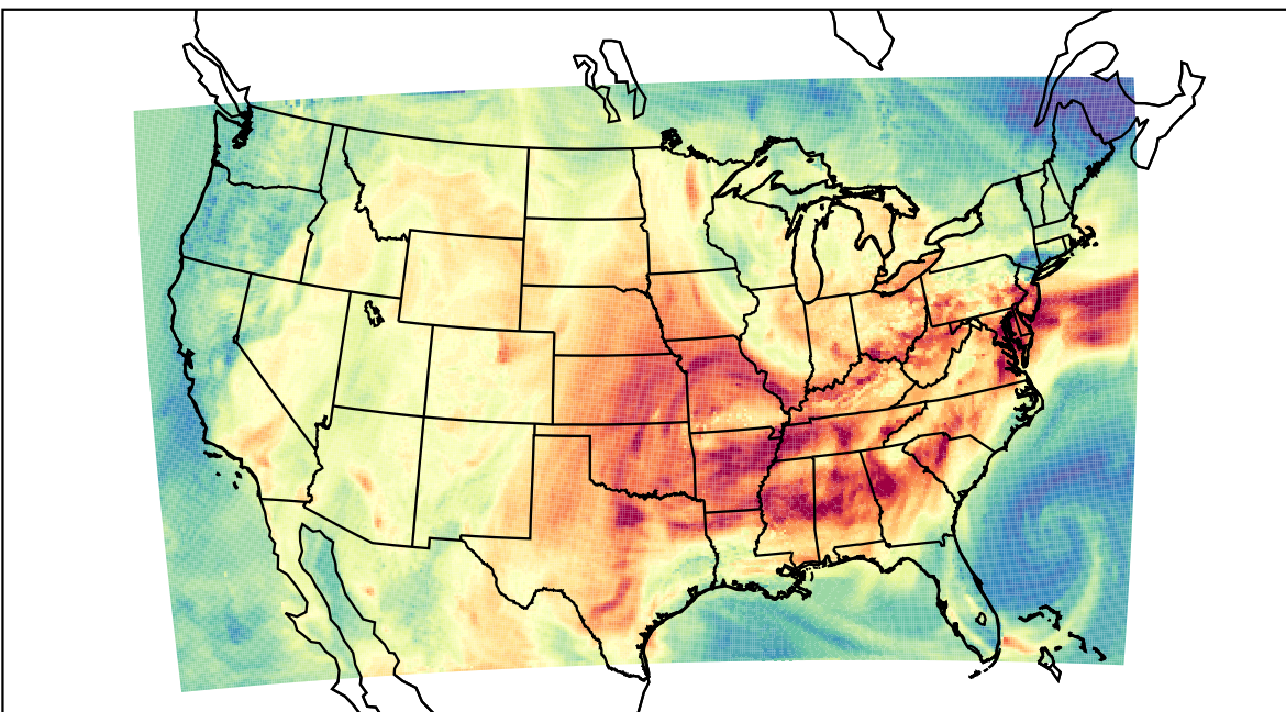
WRF (2019-09-16_21:00:00)
