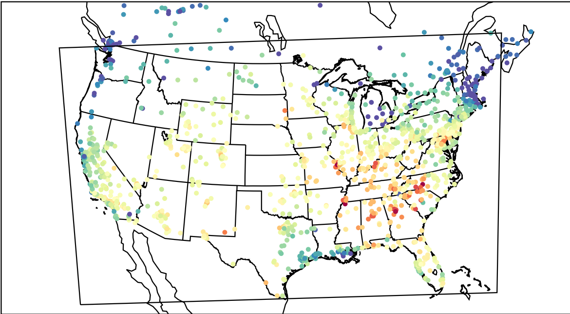
AirNOW (2019-09-17_20:00:00)
