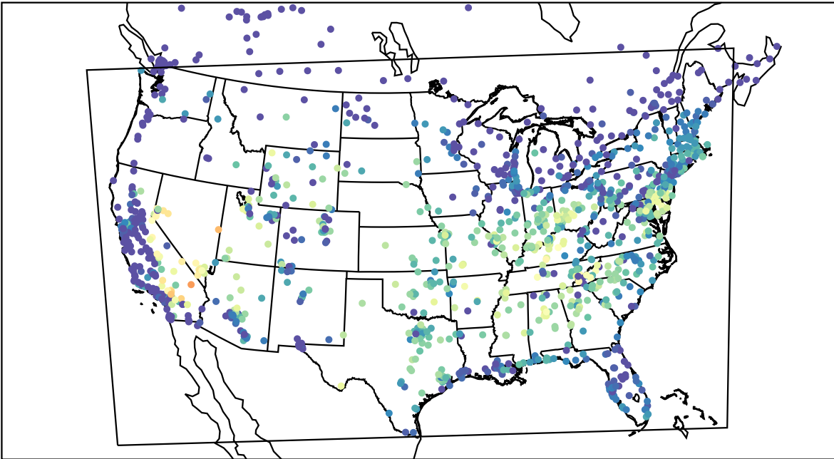
AirNOW (2019-09-16_14:00:00)
