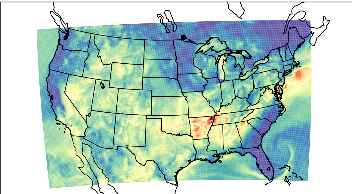
WRF (2019-09-16_09:00:00)
