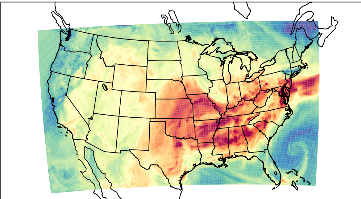
WRF (2019-09-16_19:00:00)
