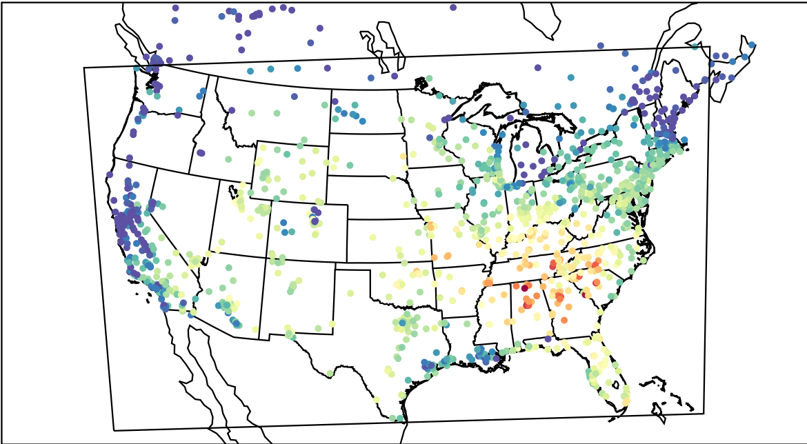
AirNOW (2019-09-17_16:00:00)
