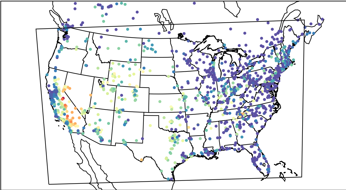
AirNOW (2019-09-16_03:00:00)
