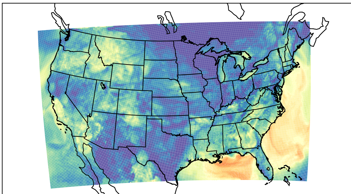
WRF (2019-09-26_12:00:00)
