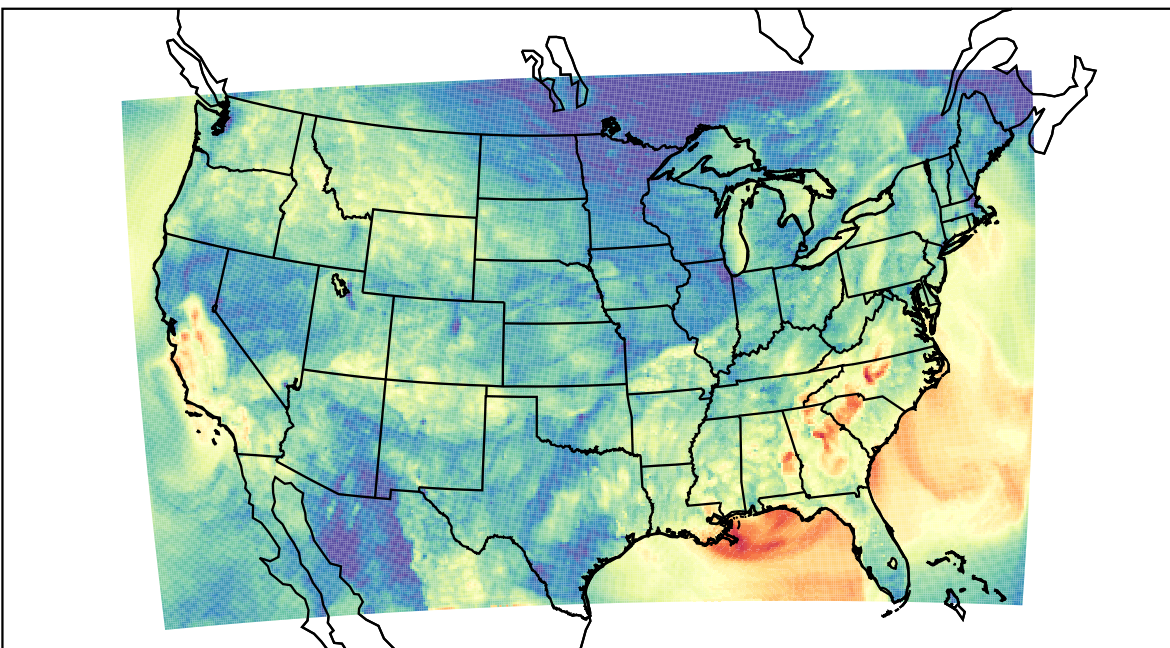
WRF (2019-09-26_03:00:00)
