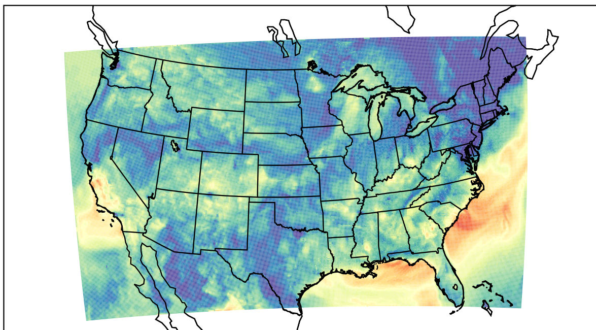
WRF (2019-09-25_06:00:00)
