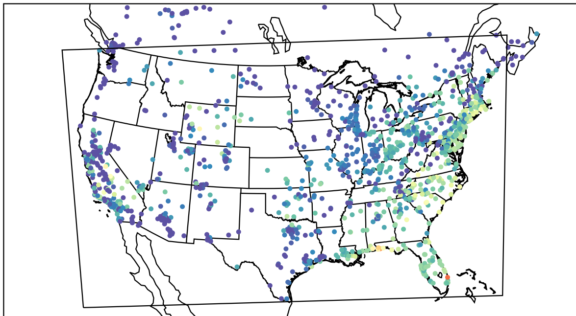
AirNOW (2019-09-26_14:00:00)
