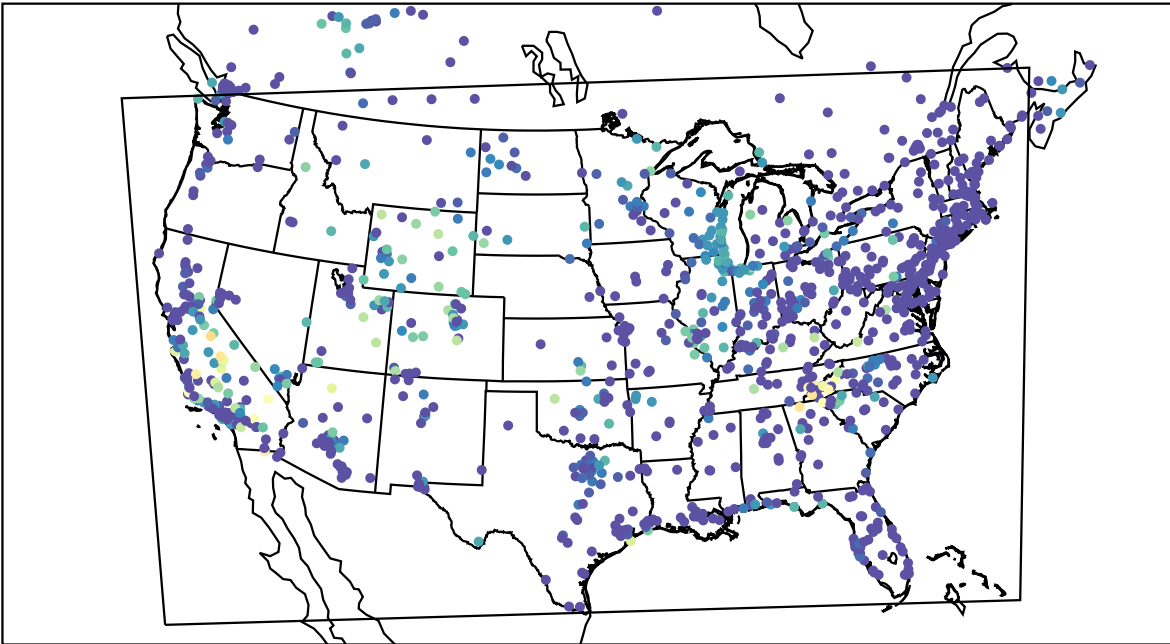
AirNOW (2019-09-25_11:00:00)
