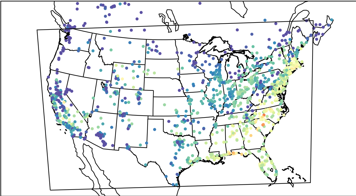
AirNOW (2019-09-26_15:00:00)
