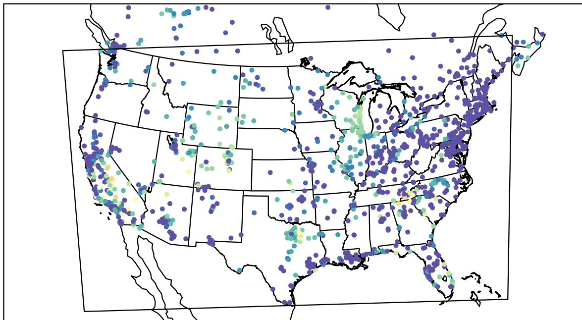
AirNOW (2019-09-25_07:00:00)
