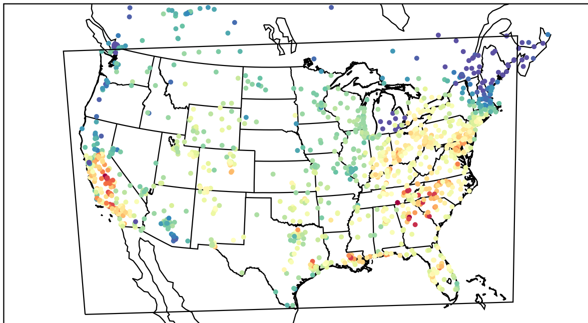
AirNOW (2019-09-25_19:00:00)
