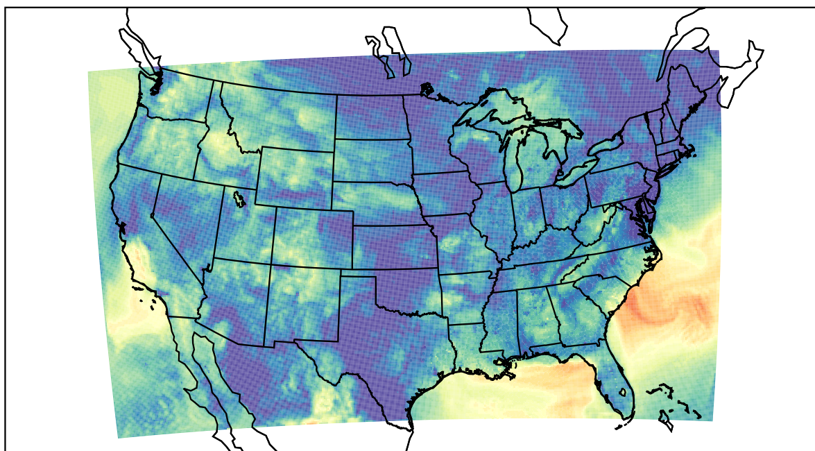
WRF (2019-09-25_13:00:00)
