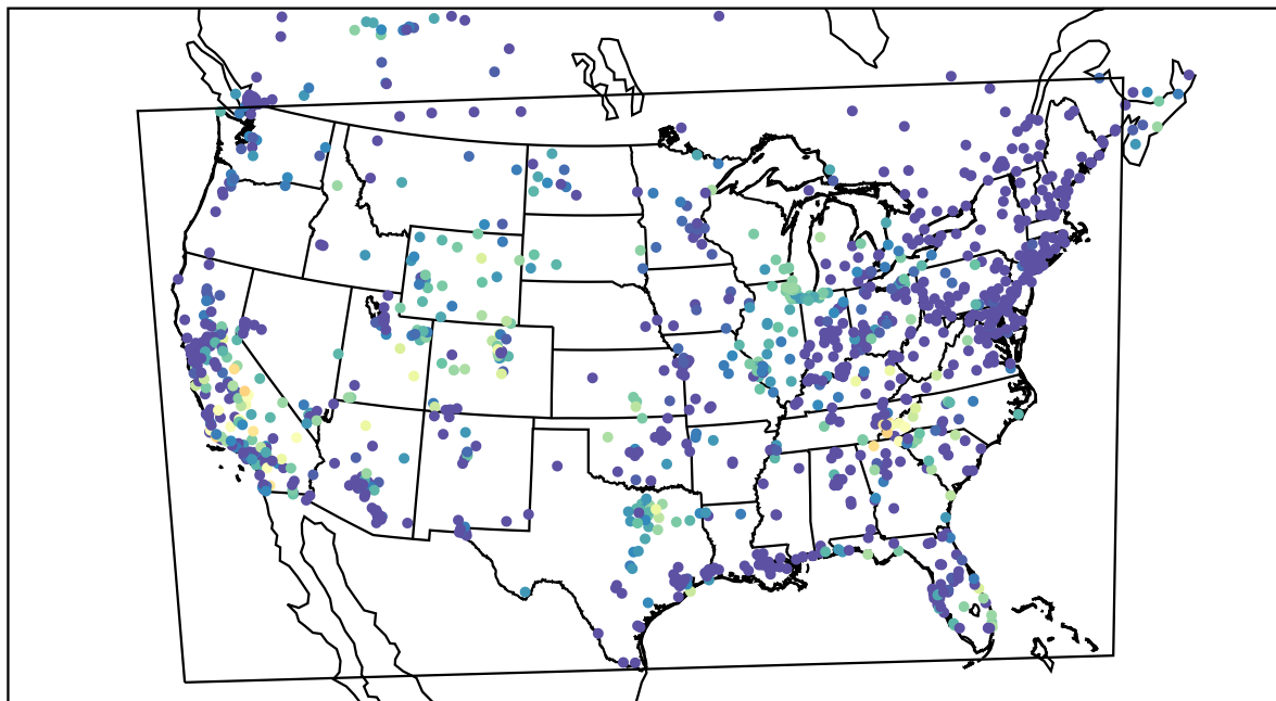
AirNOW (2019-09-25_08:00:00)
