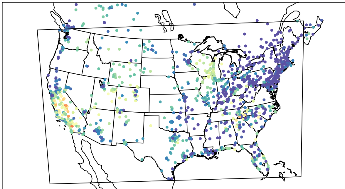
AirNOW (2019-09-25_02:00:00)
