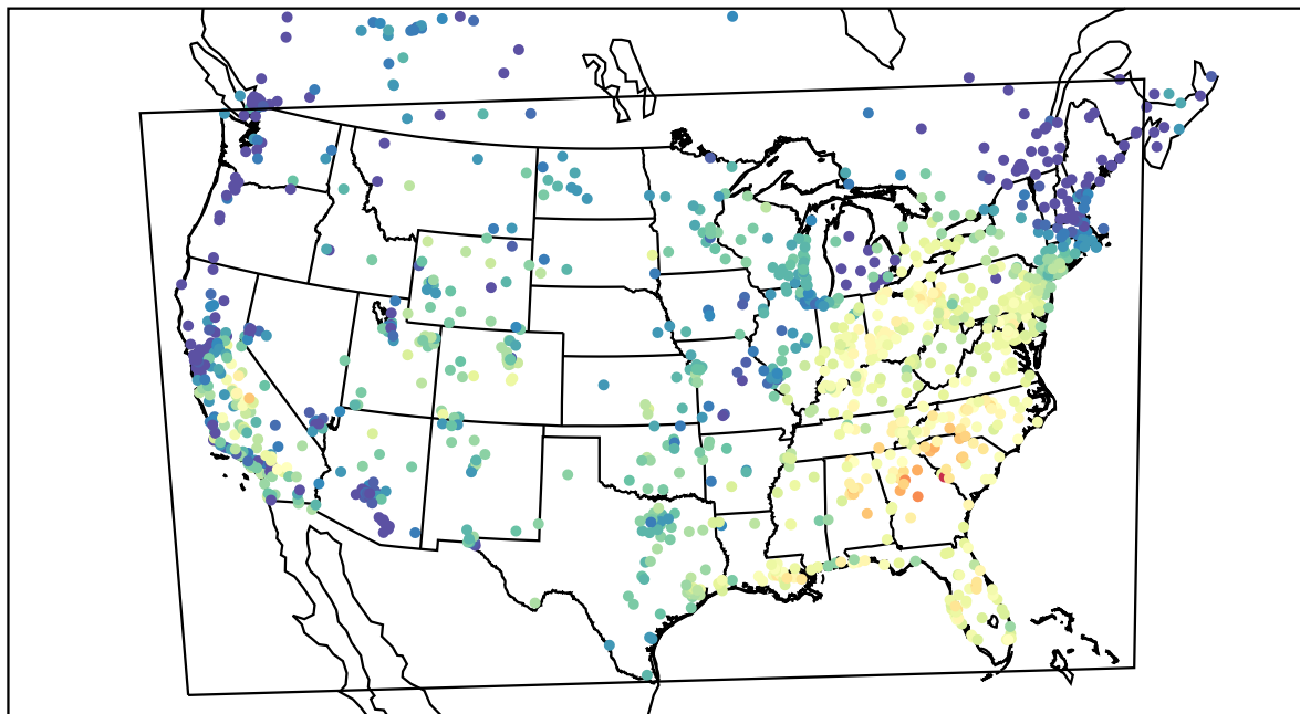
AirNOW (2019-09-25_16:00:00)
