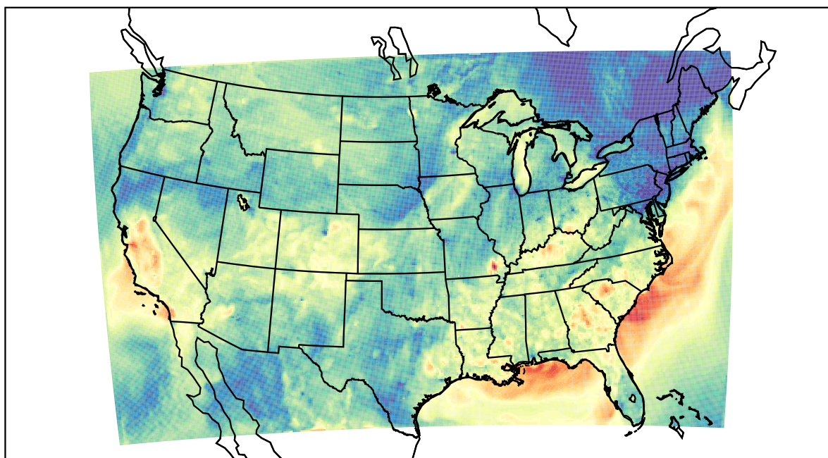
WRF (2019-09-25_01:00:00)
