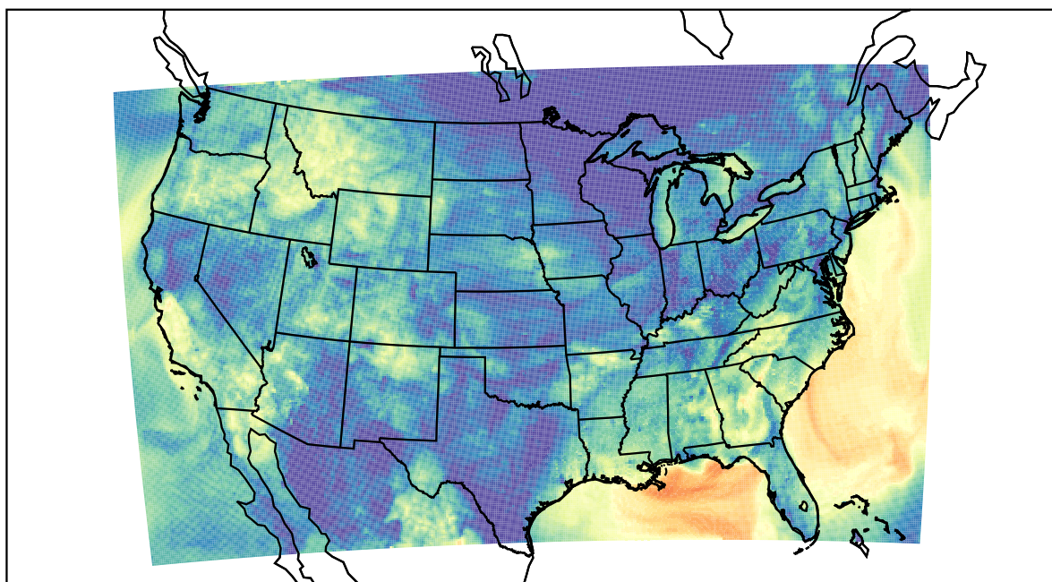
WRF (2019-09-26_11:00:00)
