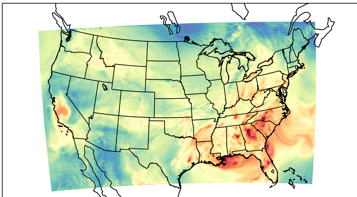
WRF (2019-09-25_19:00:00)
