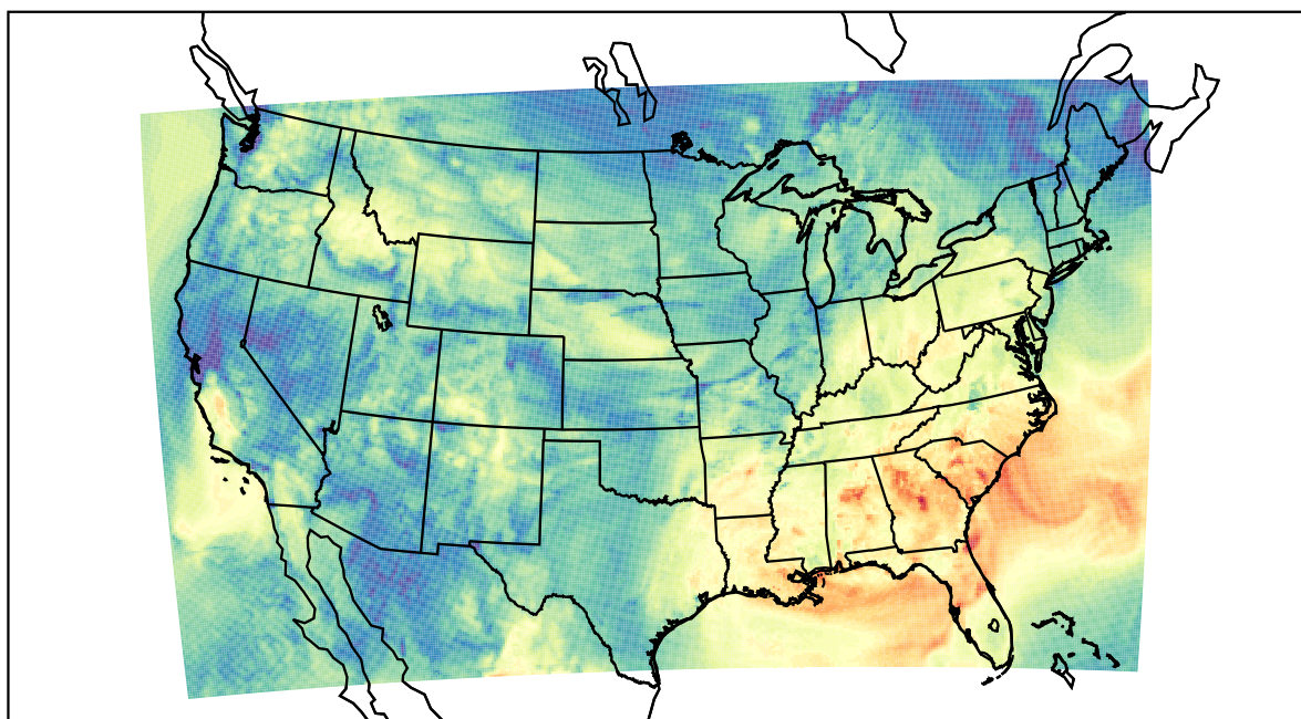
WRF (2019-09-25_16:00:00)
