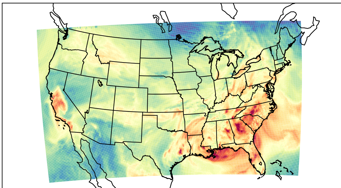
WRF (2019-09-25_21:00:00)
