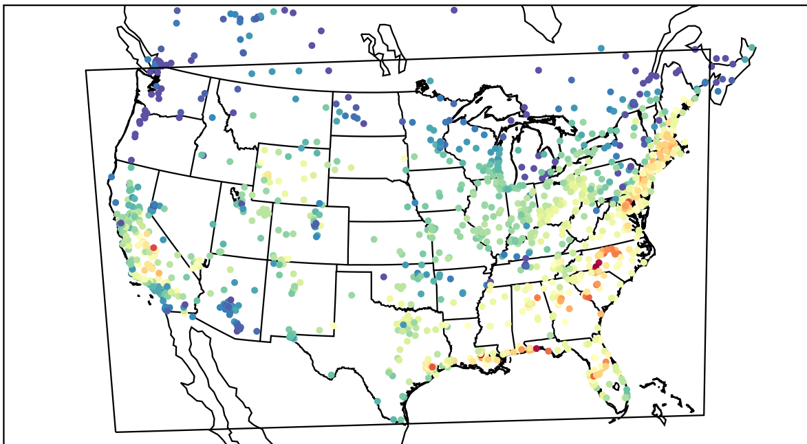
AirNOW (2019-09-26_17:00:00)
