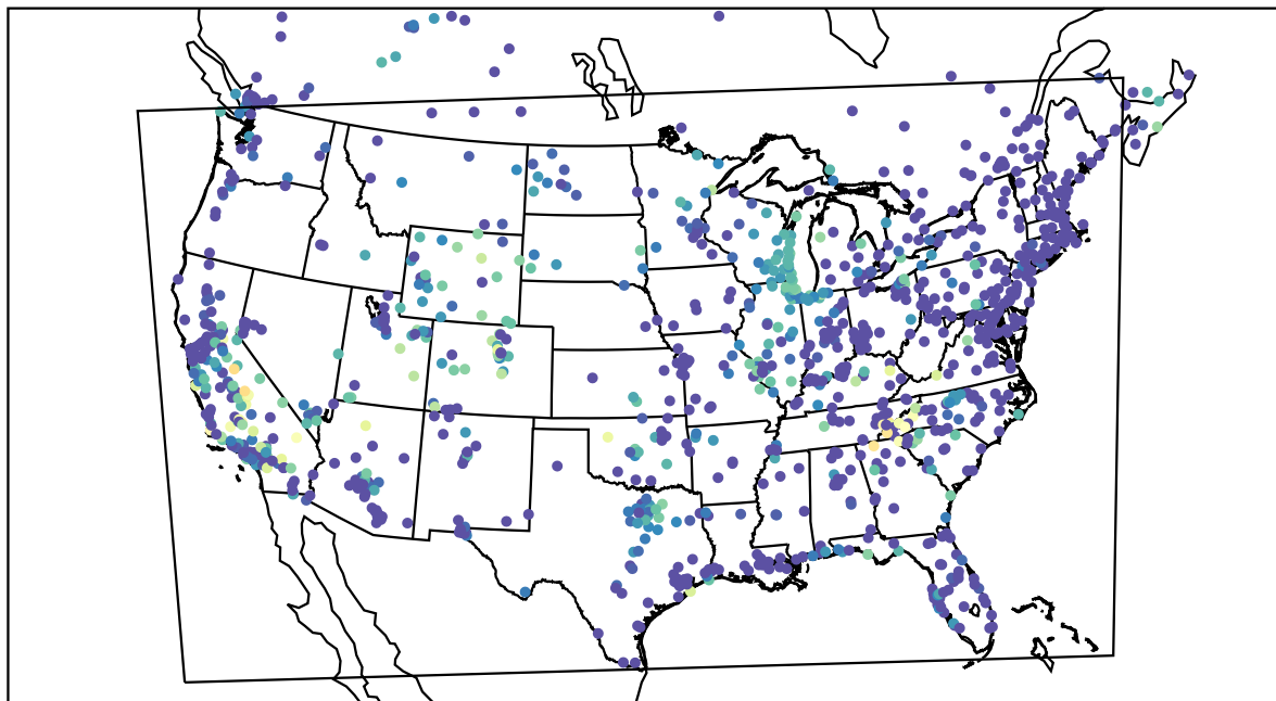
AirNOW (2019-09-25_10:00:00)
