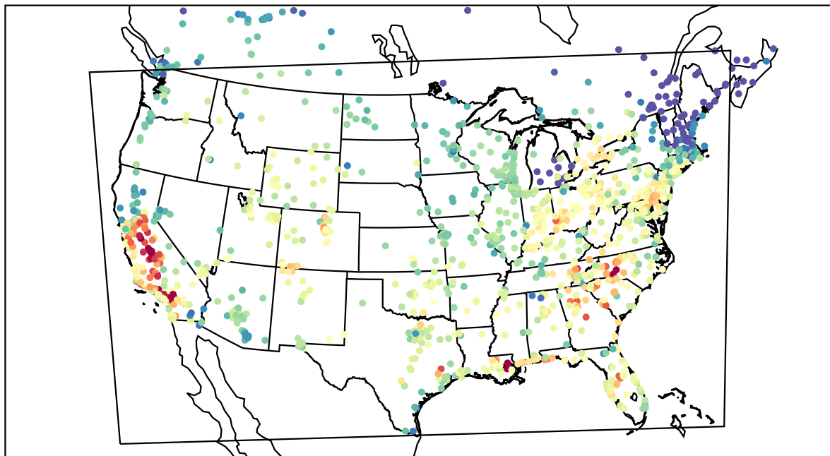
AirNOW (2019-09-25_22:00:00)
