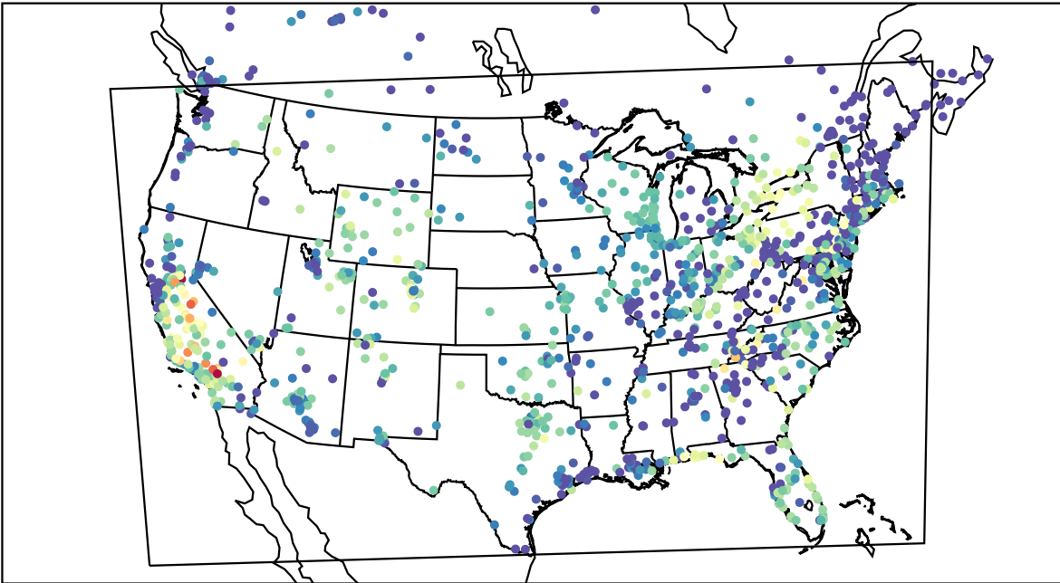
AirNOW (2019-09-26_03:00:00)
