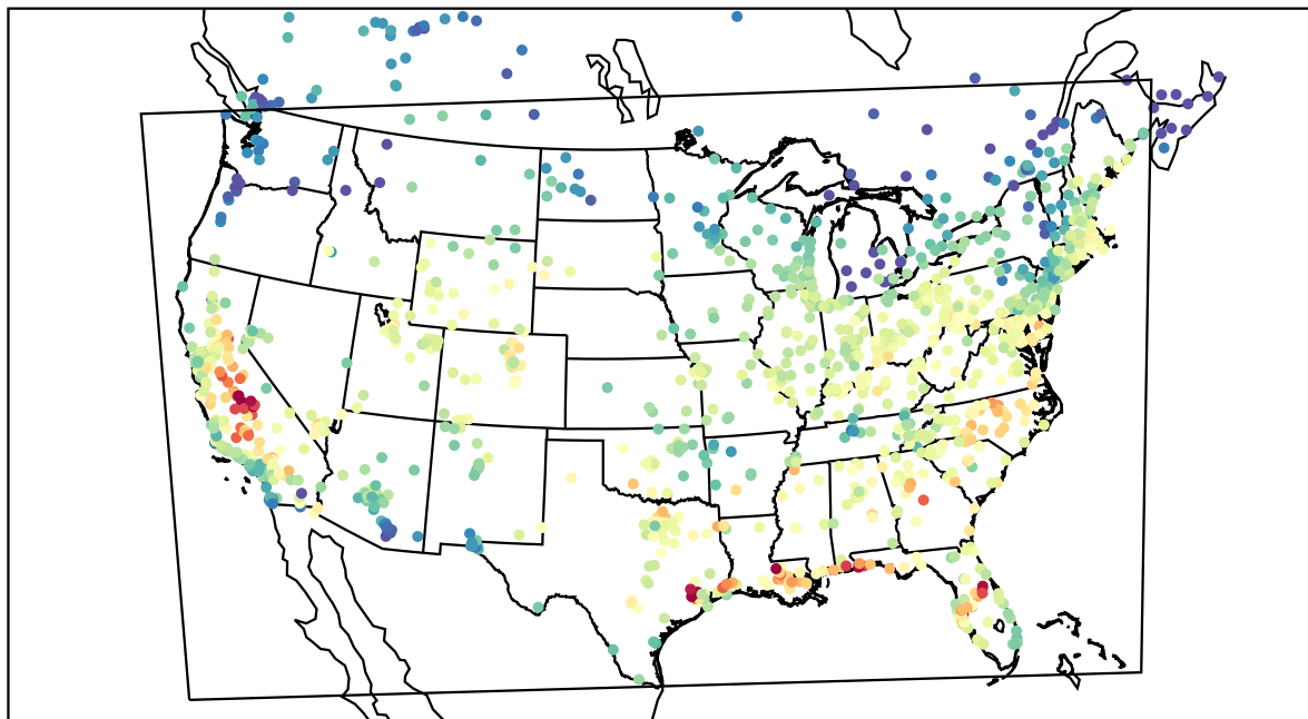
AirNOW (2019-09-26_21:00:00)
