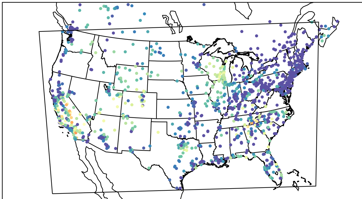
AirNOW (2019-09-25_03:00:00)
