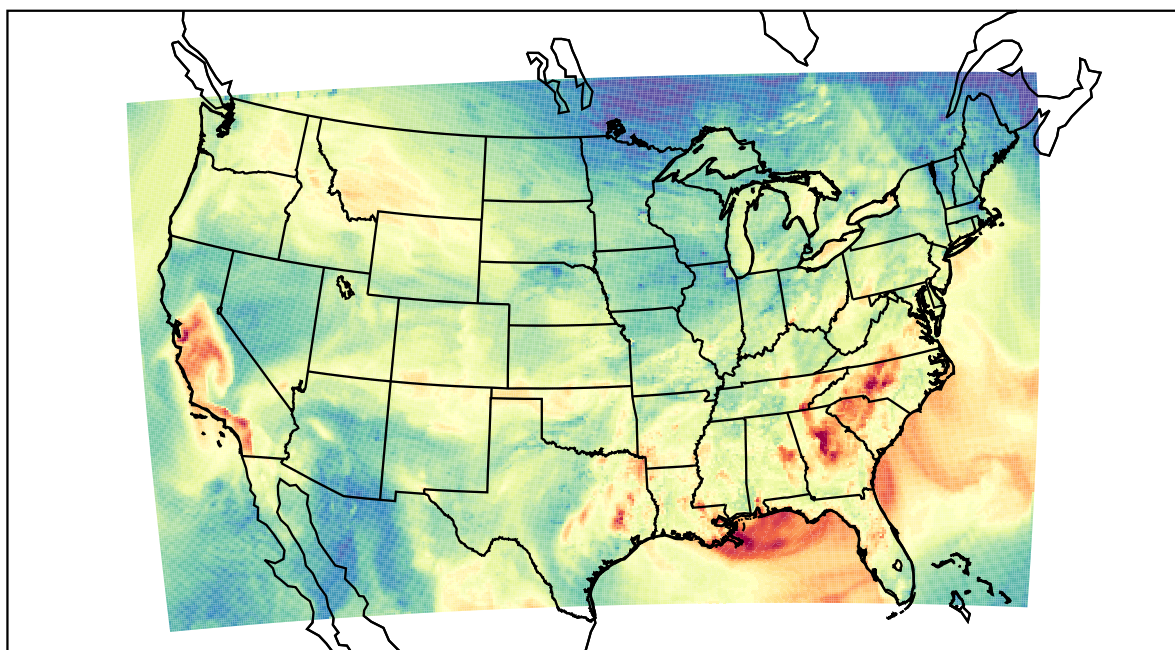
WRF (2019-09-25_23:00:00)
