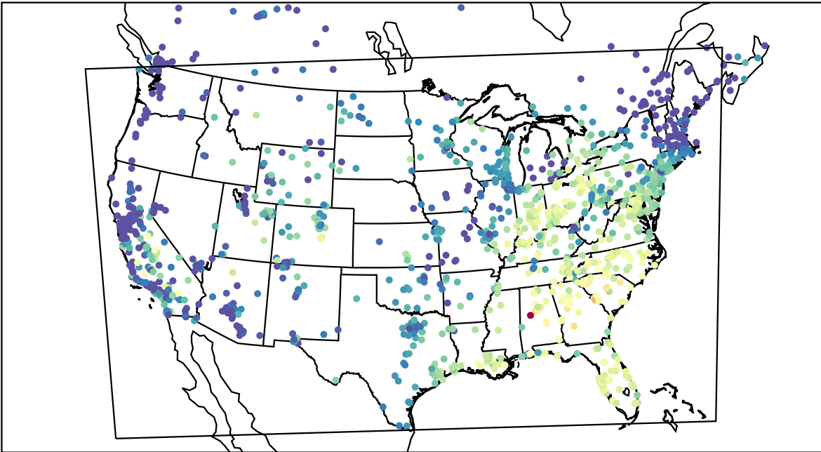
AirNOW (2019-09-25_15:00:00)
