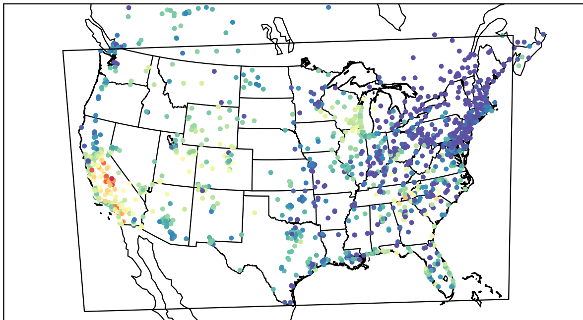
AirNOW (2019-09-25_01:00:00)
