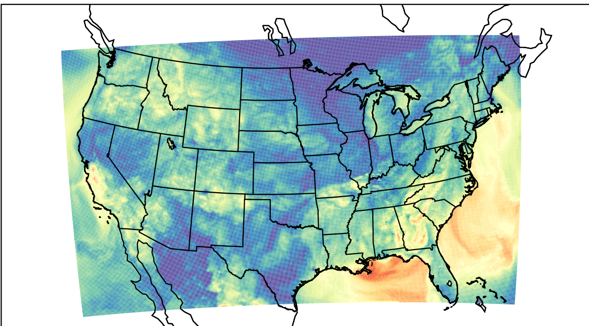
WRF (2019-09-26_07:00:00)
