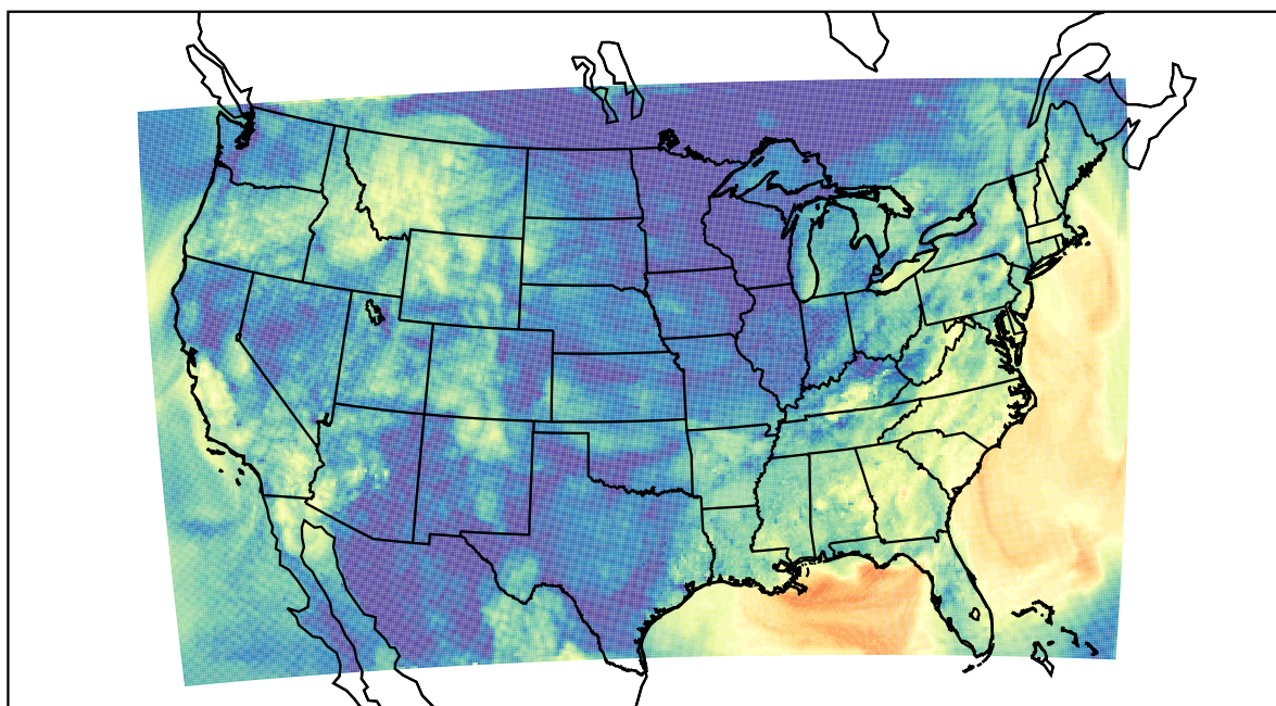
WRF (2019-09-26_14:00:00)
