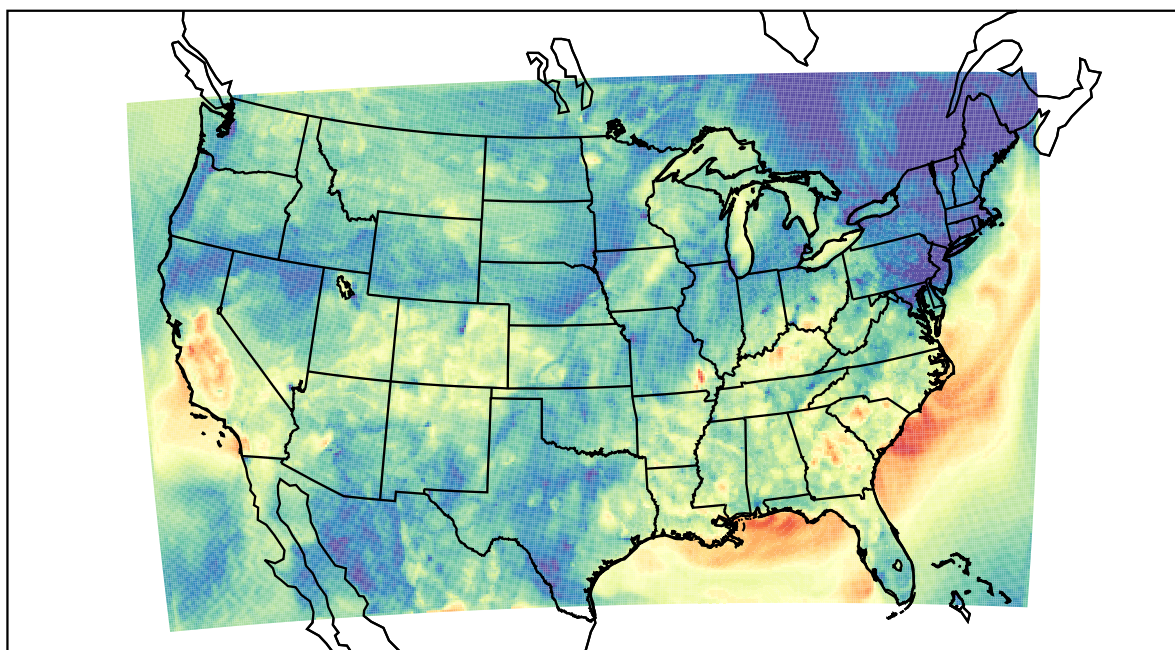
WRF (2019-09-25_02:00:00)
