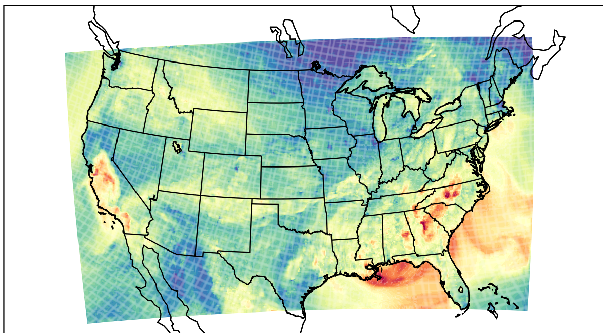
WRF (2019-09-26_01:00:00)
