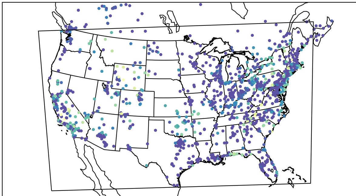
AirNOW (2019-09-26_12:00:00)
