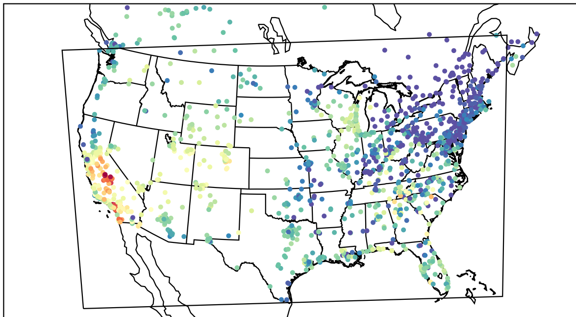
AirNOW (2019-09-25_00:00:00)
