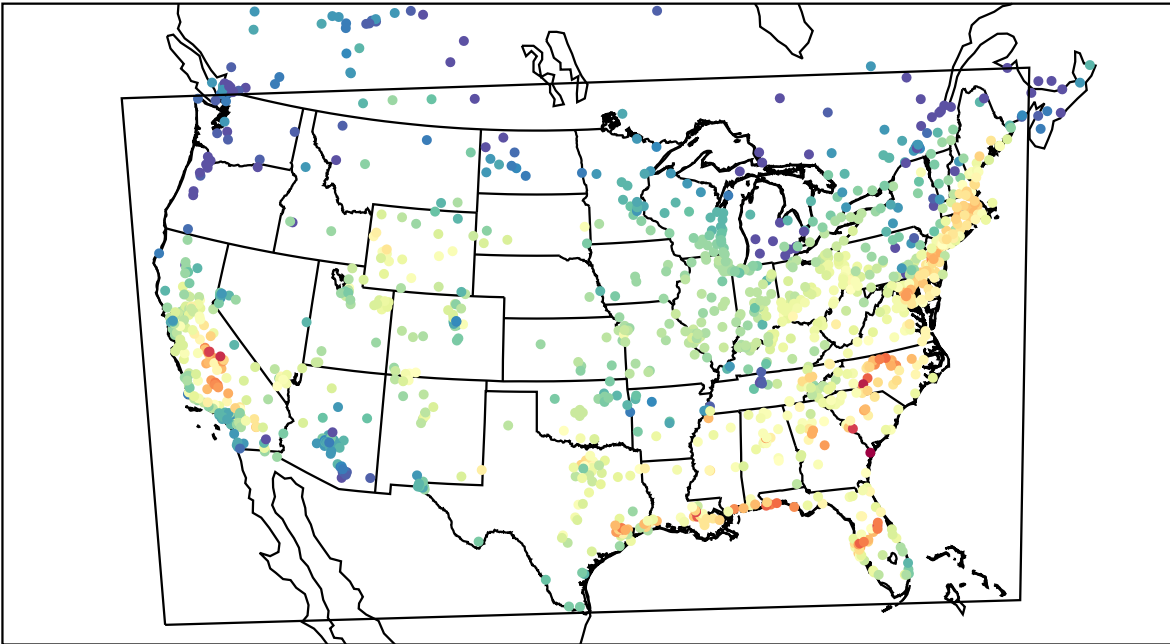
AirNOW (2019-09-26_18:00:00)
