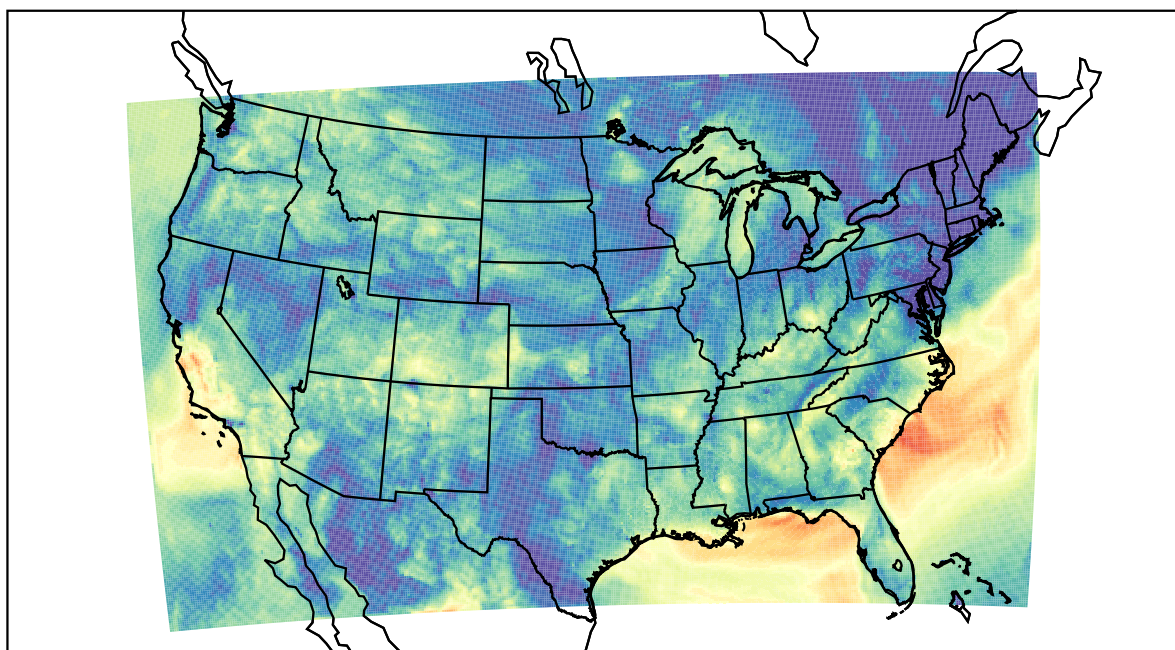
WRF (2019-09-25_07:00:00)
