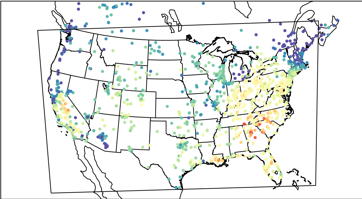
AirNOW (2019-09-25_17:00:00)
