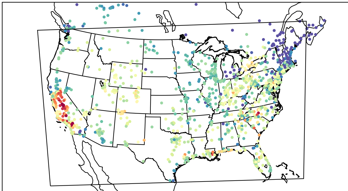
AirNOW (2019-09-25_23:00:00)
