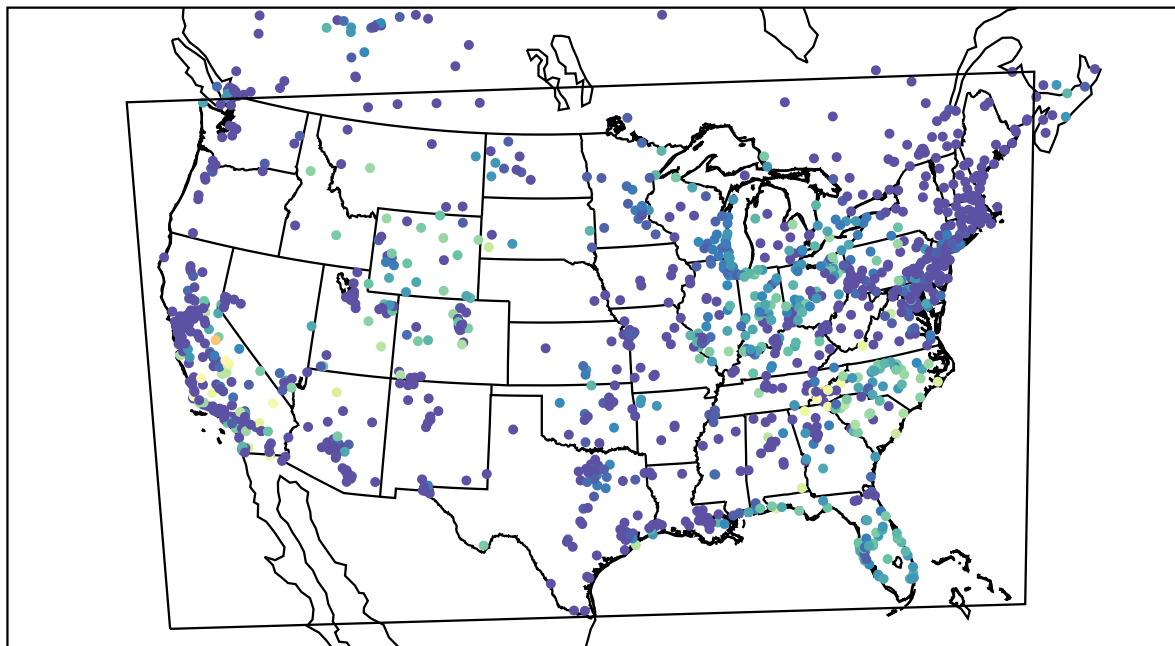
AirNOW (2019-09-25_13:00:00)
