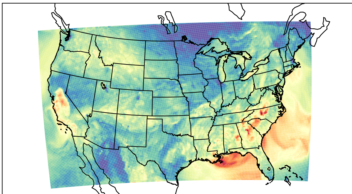
WRF (2019-09-26_02:00:00)
