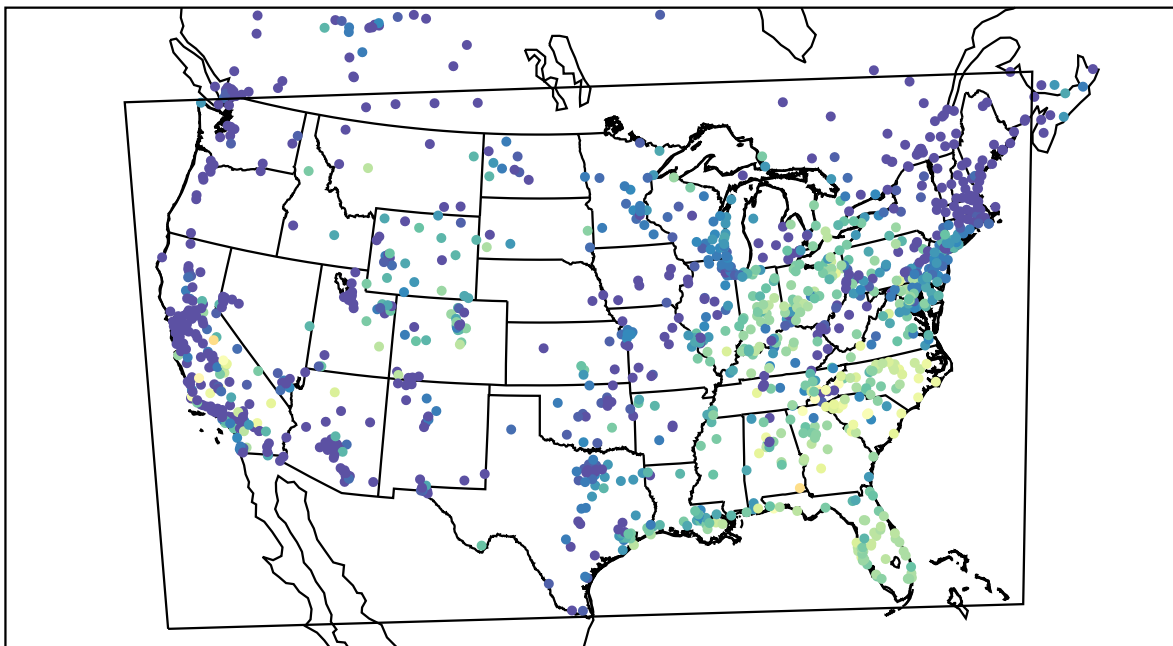
AirNOW (2019-09-25_14:00:00)
