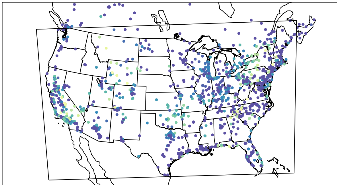
AirNOW (2019-09-26_10:00:00)
