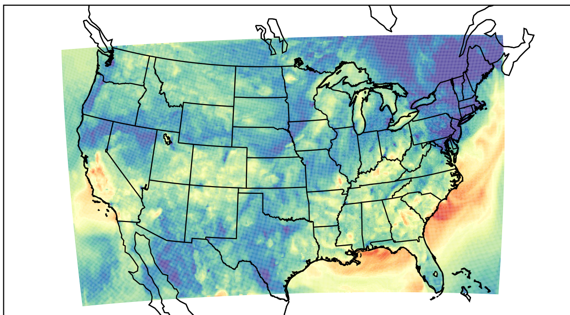
WRF (2019-09-25_03:00:00)
