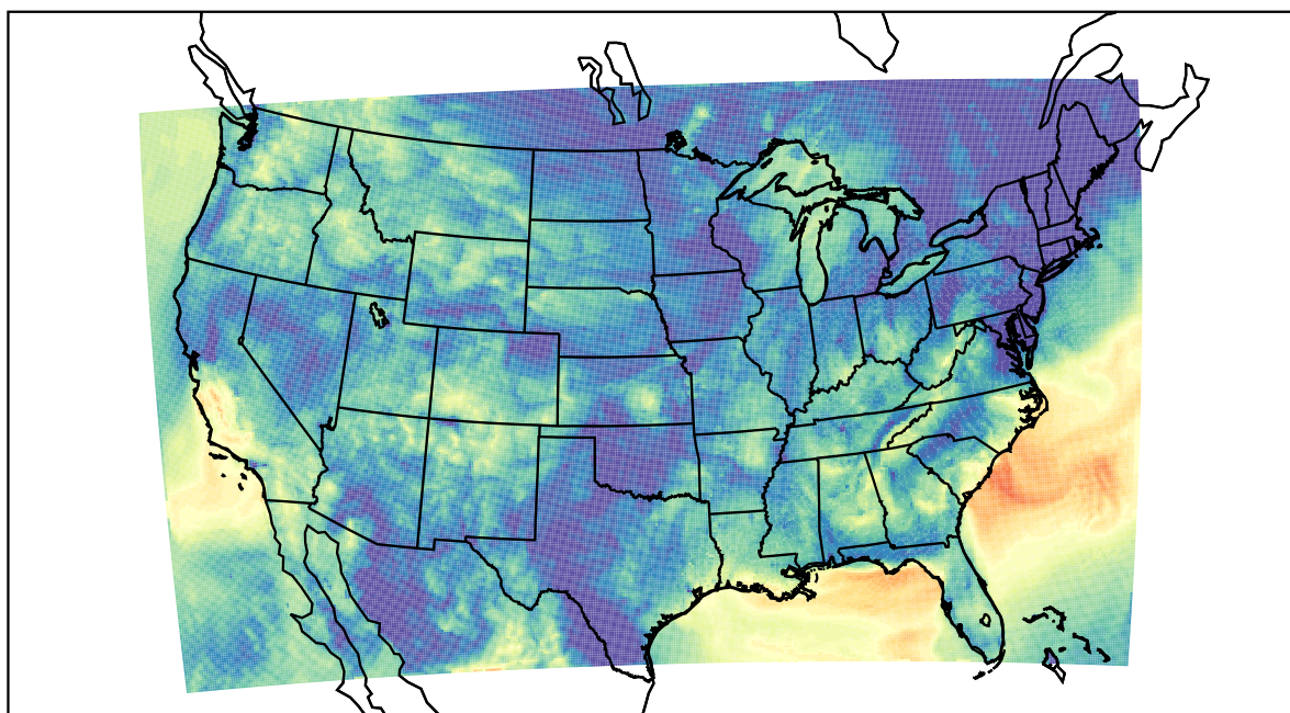
WRF (2019-09-25_10:00:00)
