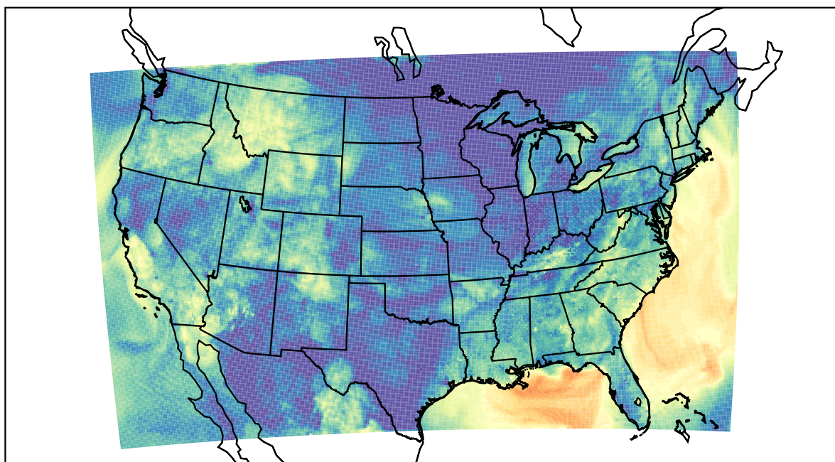
WRF (2019-09-26_13:00:00)
