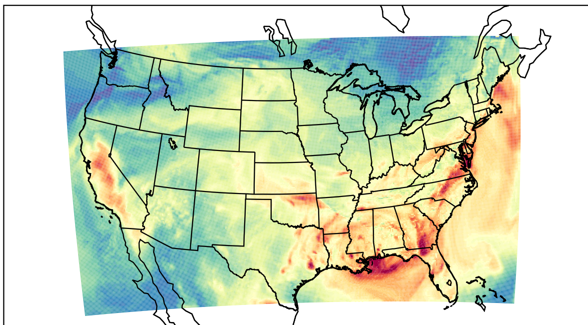
WRF (2019-09-26_21:00:00)
