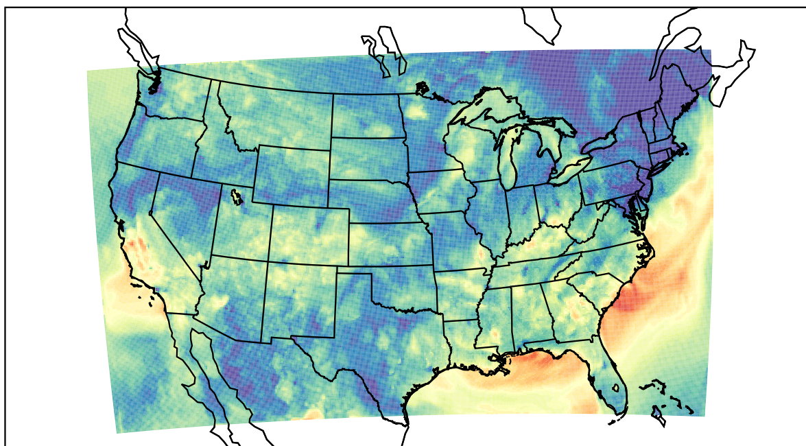
WRF (2019-09-25_04:00:00)
