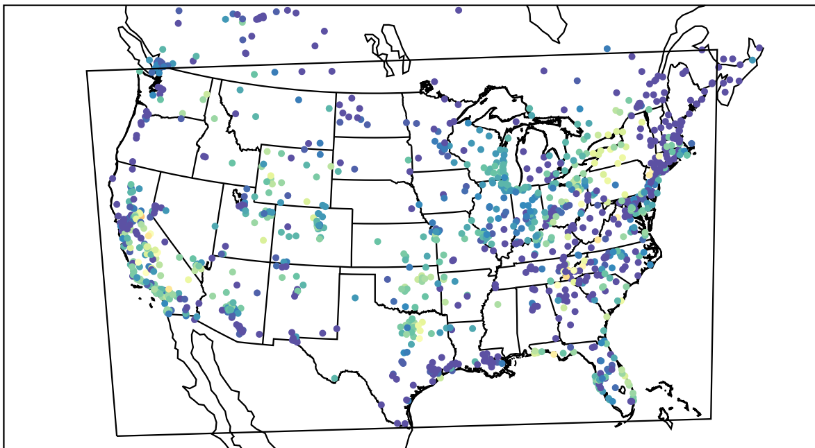
AirNOW (2019-09-26_06:00:00)
