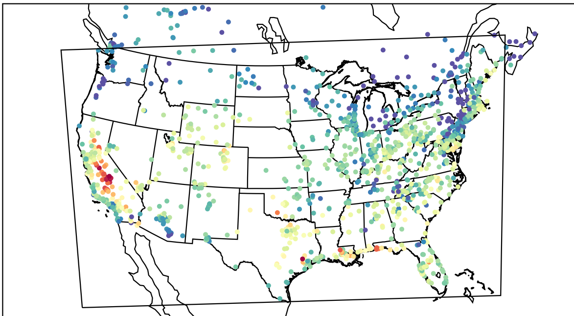
AirNOW (2019-09-26_23:00:00)
