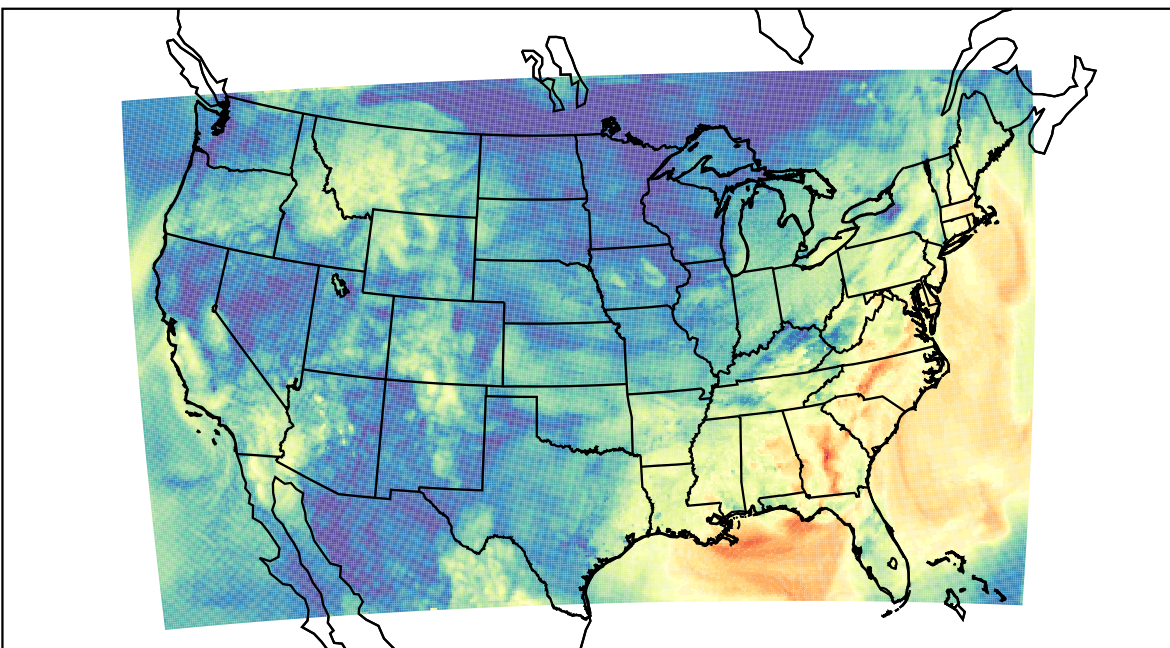
WRF (2019-09-26_15:00:00)
