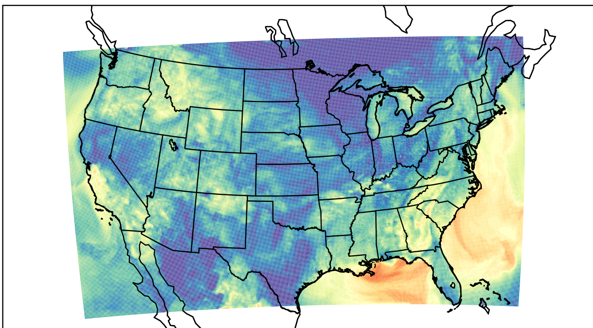
WRF (2019-09-26_09:00:00)
