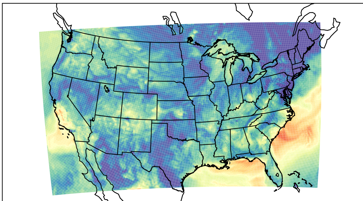
WRF (2019-09-25_08:00:00)
