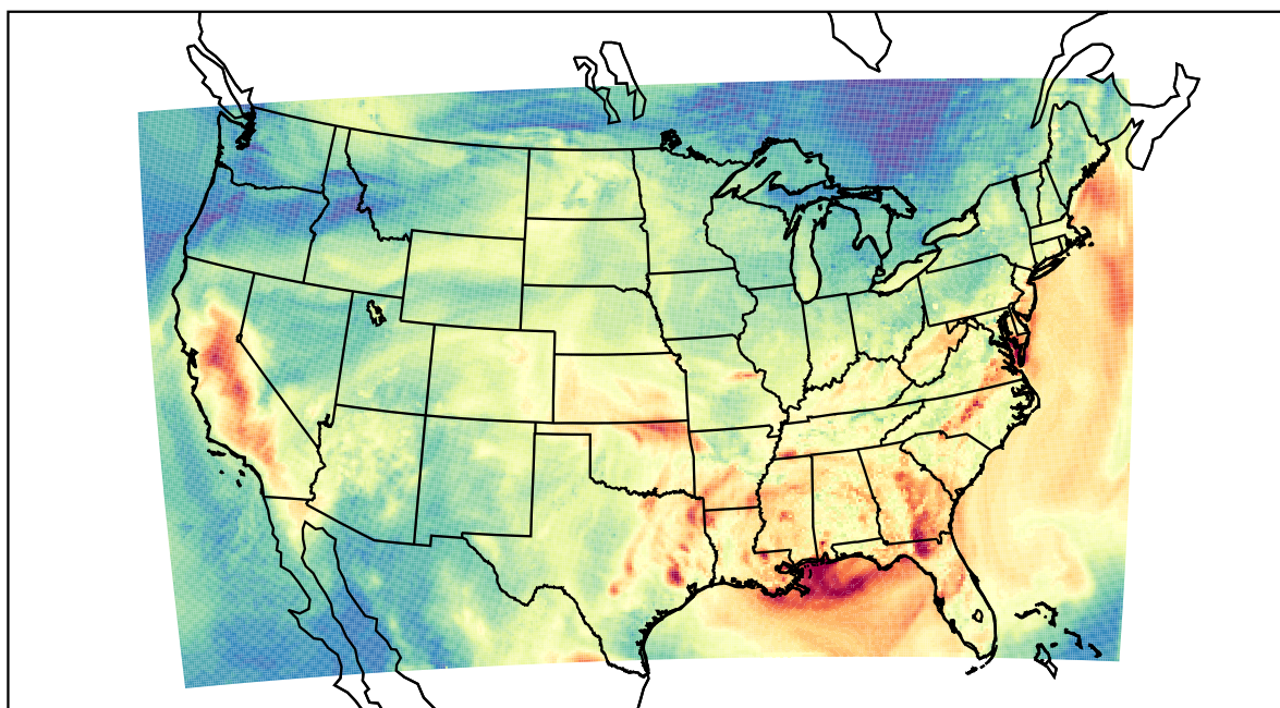
WRF (2019-09-26_22:00:00)
