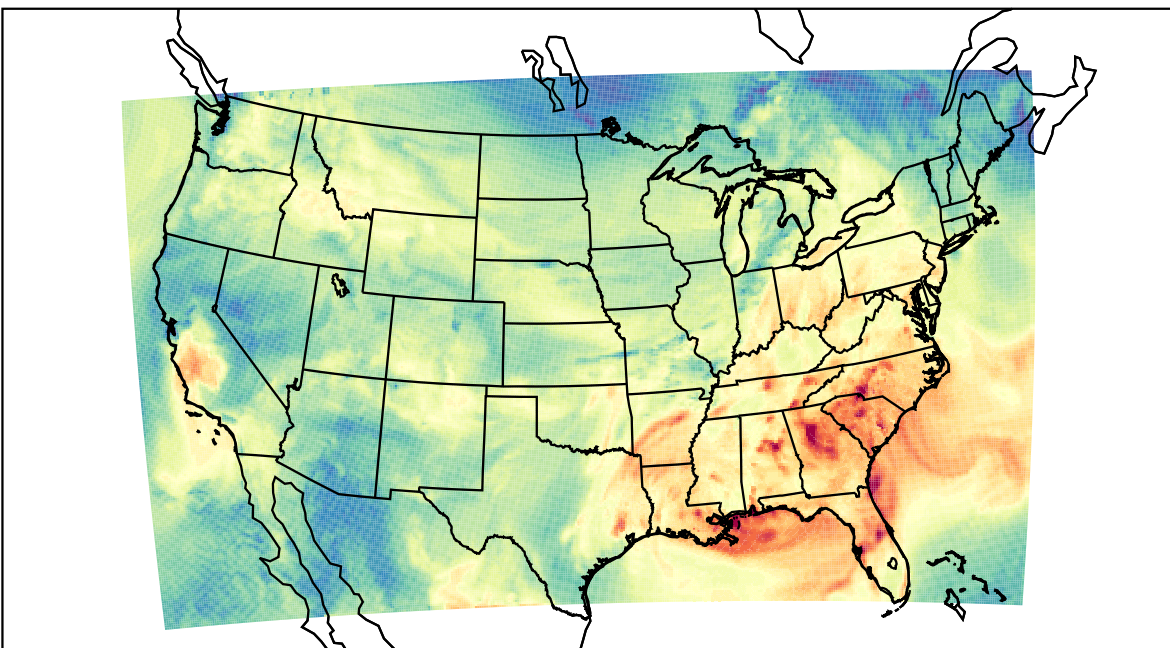
WRF (2019-09-25_18:00:00)
