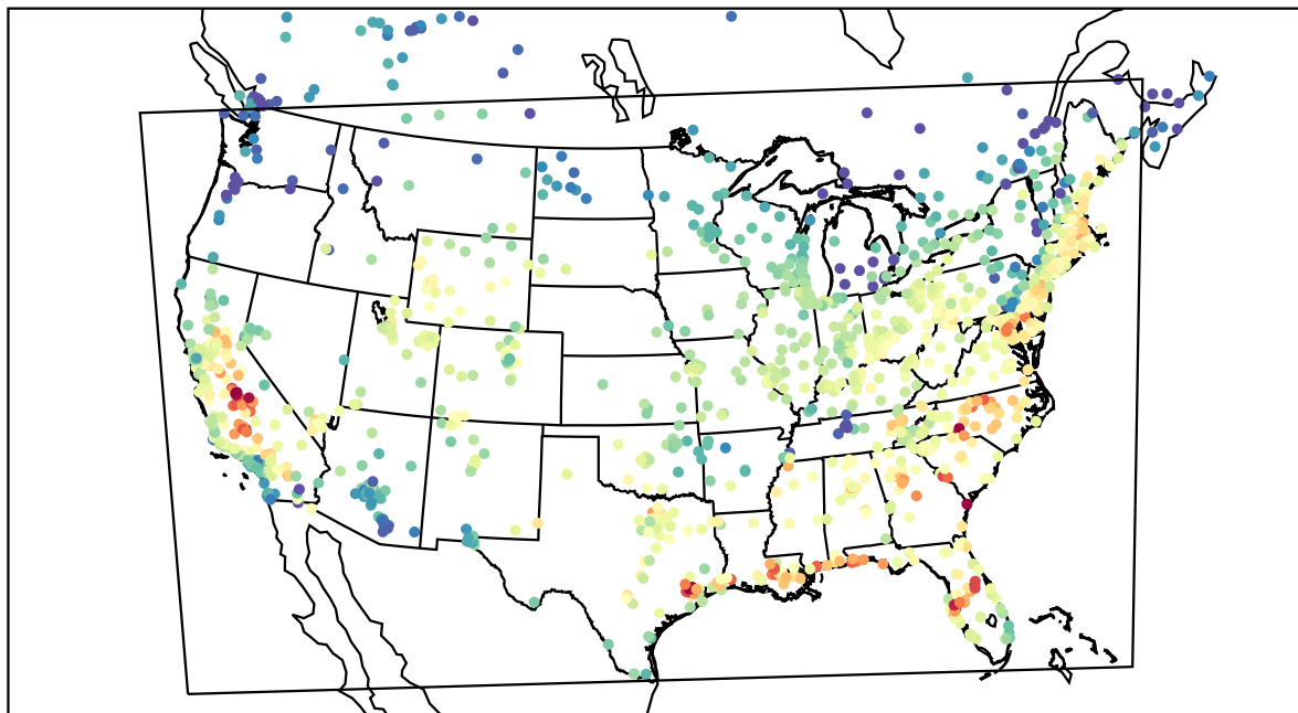
AirNOW (2019-09-26_19:00:00)
