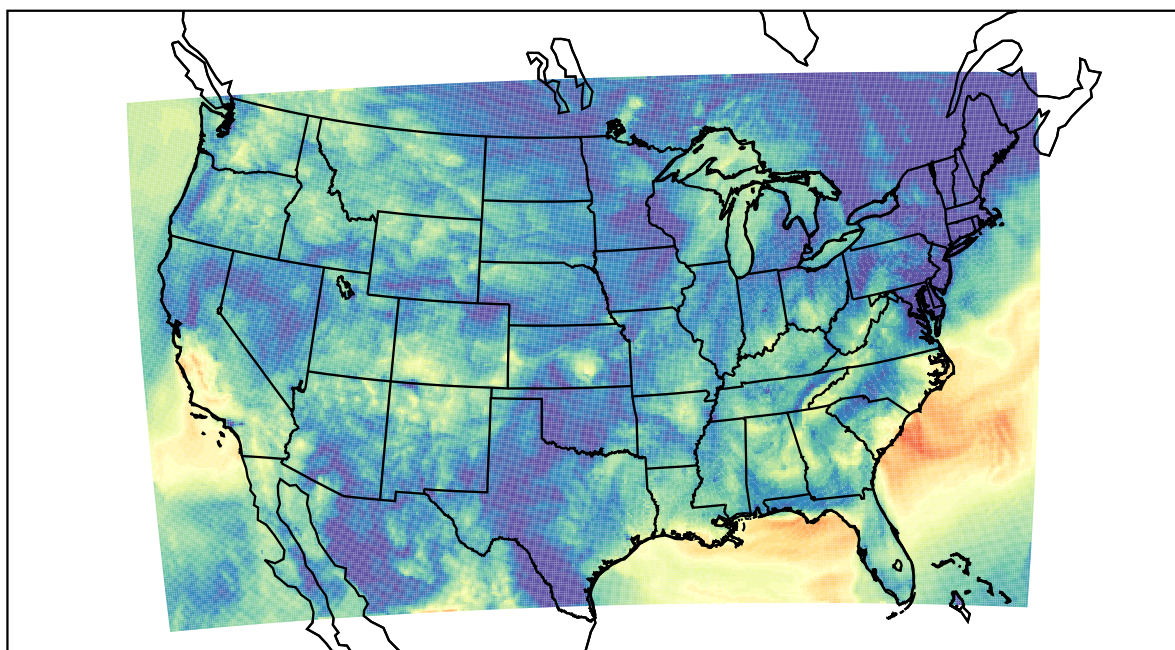
WRF (2019-09-25_09:00:00)
