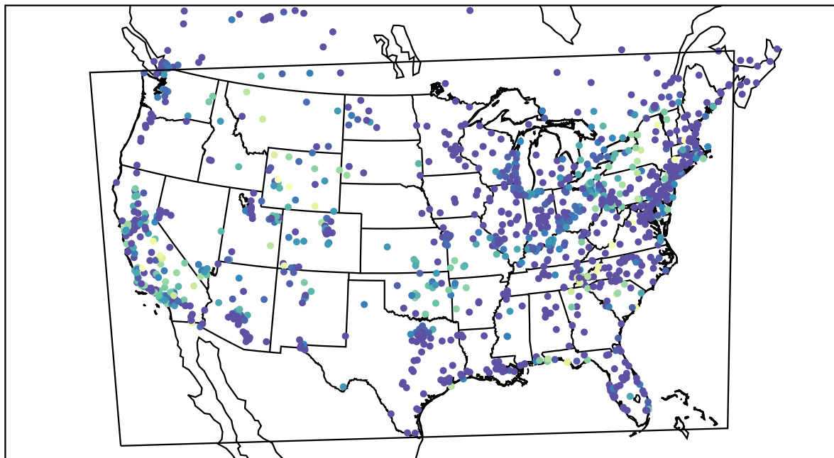
AirNOW (2019-09-26_11:00:00)
