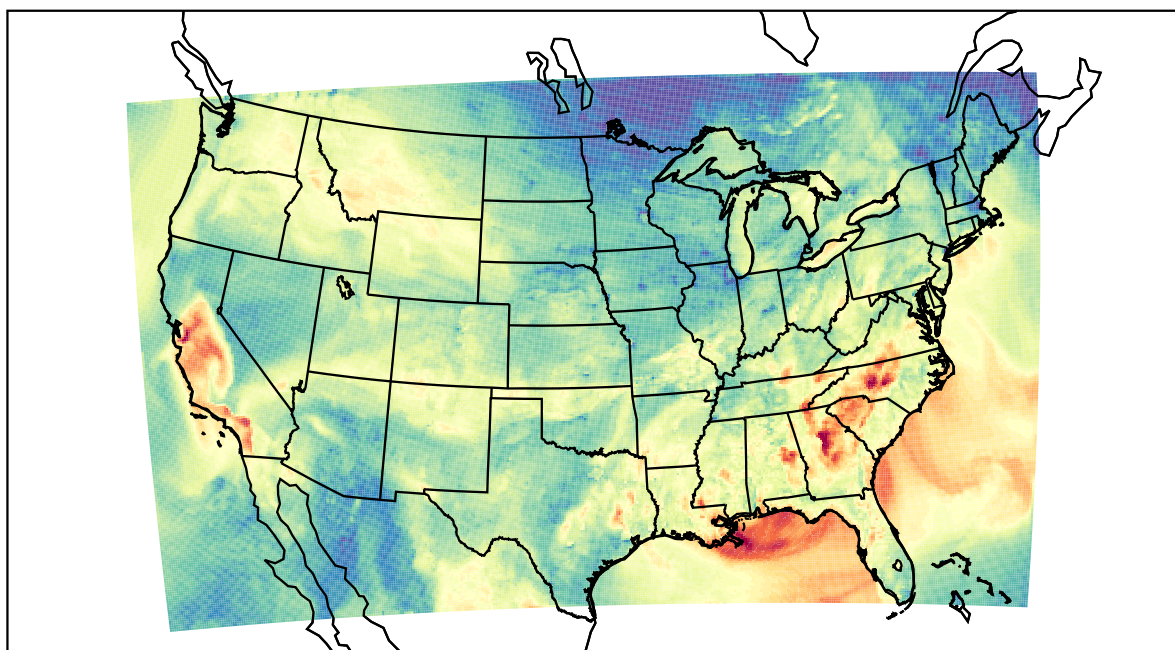
WRF (2019-09-26_00:00:00)
