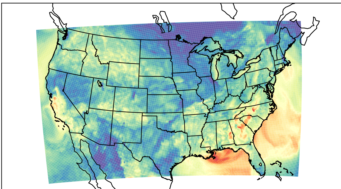
WRF (2019-09-26_04:00:00)
