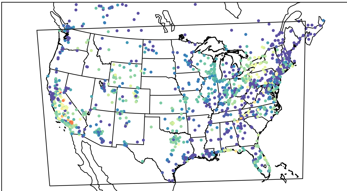
AirNOW (2019-09-26_04:00:00)
