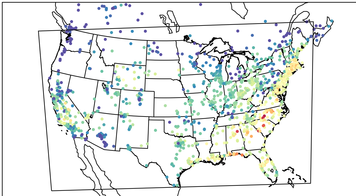
AirNOW (2019-09-26_16:00:00)
