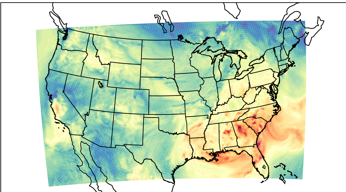
WRF (2019-09-25_17:00:00)
