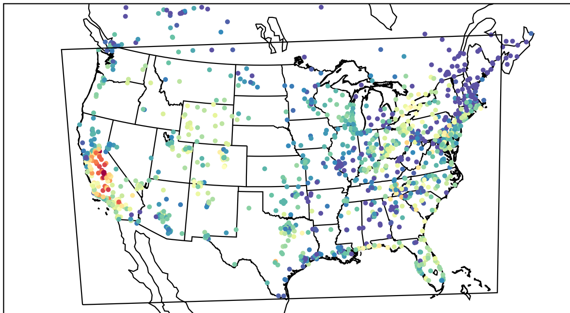
AirNOW (2019-09-26_01:00:00)
