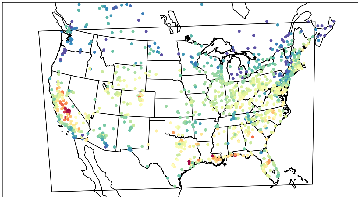
AirNOW (2019-09-26_22:00:00)
