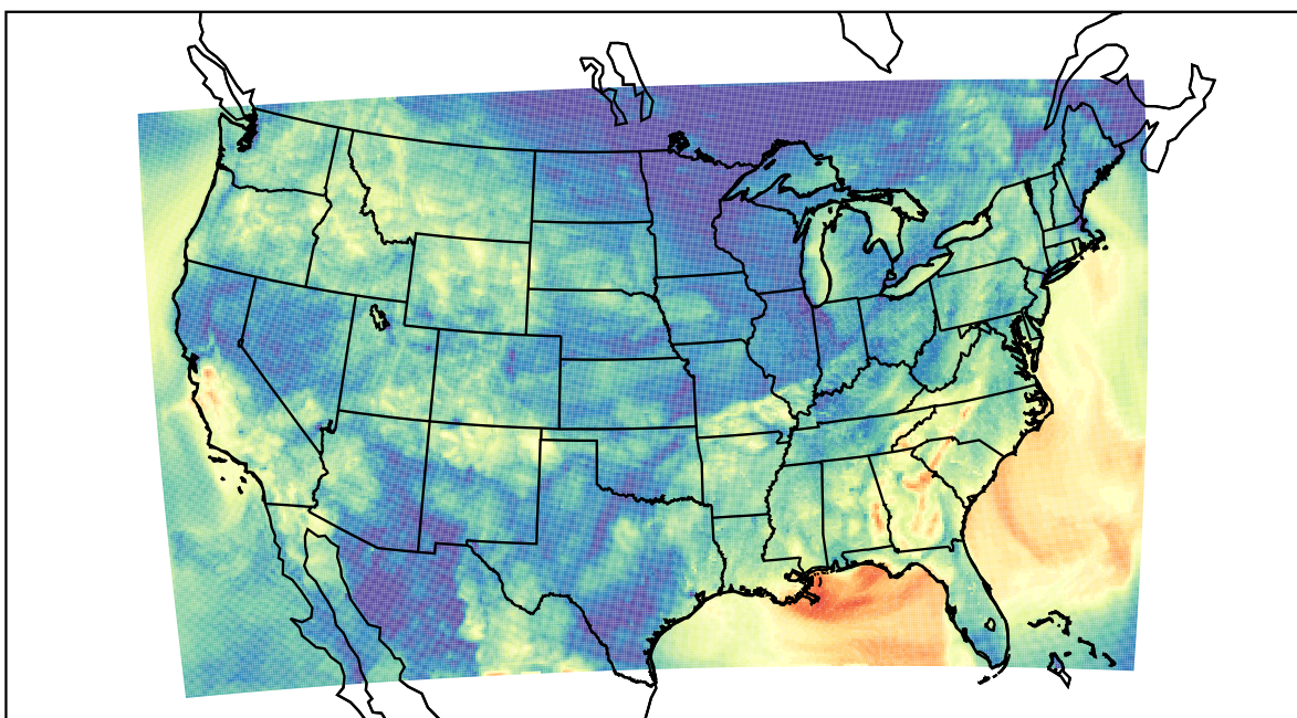
WRF (2019-09-26_06:00:00)
