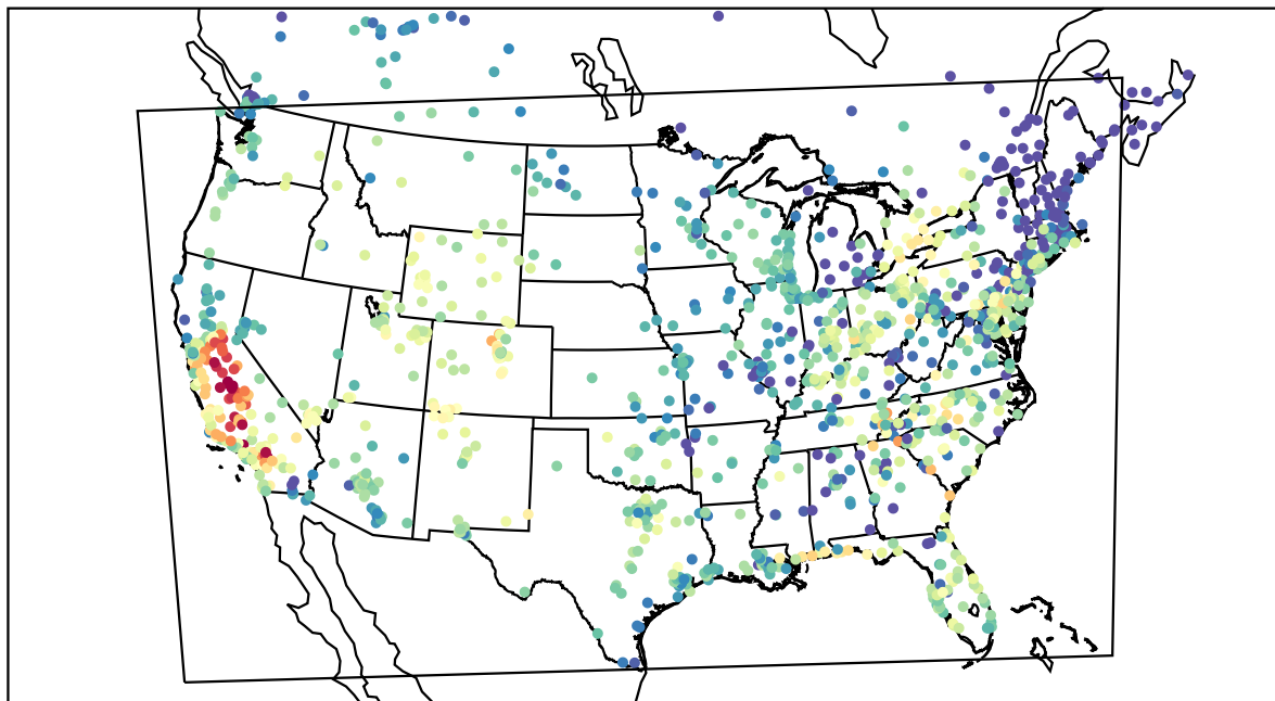
AirNOW (2019-09-26_00:00:00)
