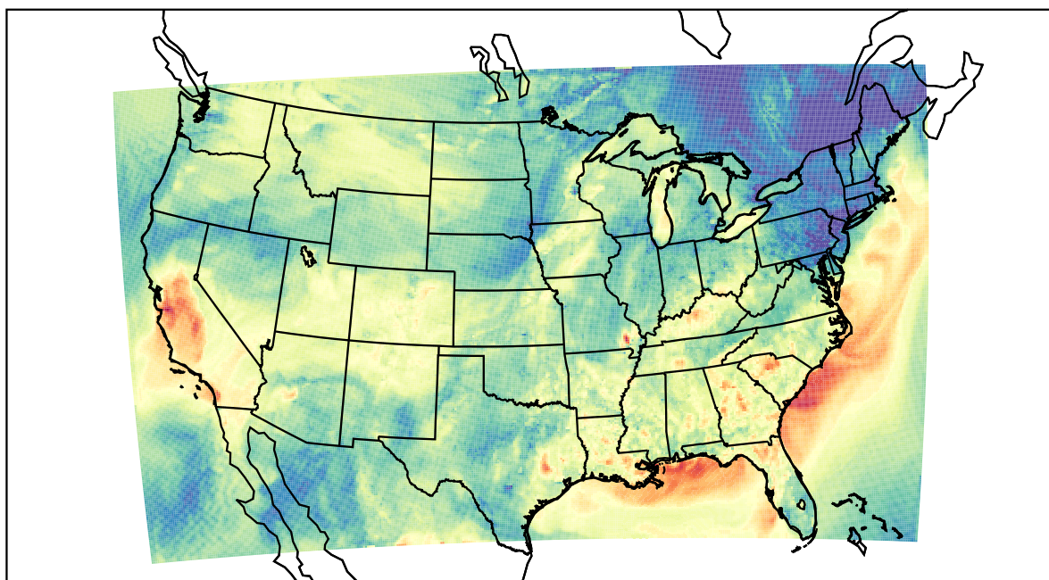
WRF (2019-09-25_00:00:00)
