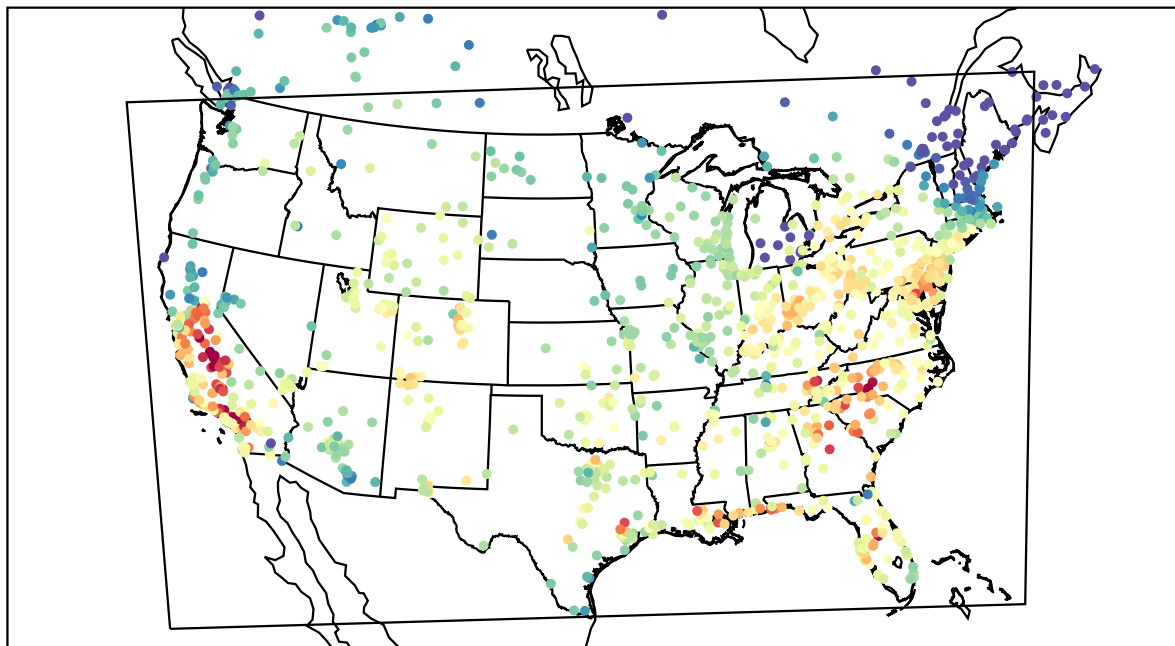
AirNOW (2019-09-25_21:00:00)
