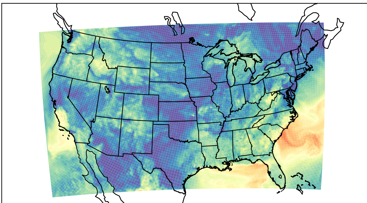
WRF (2019-09-25_14:00:00)
