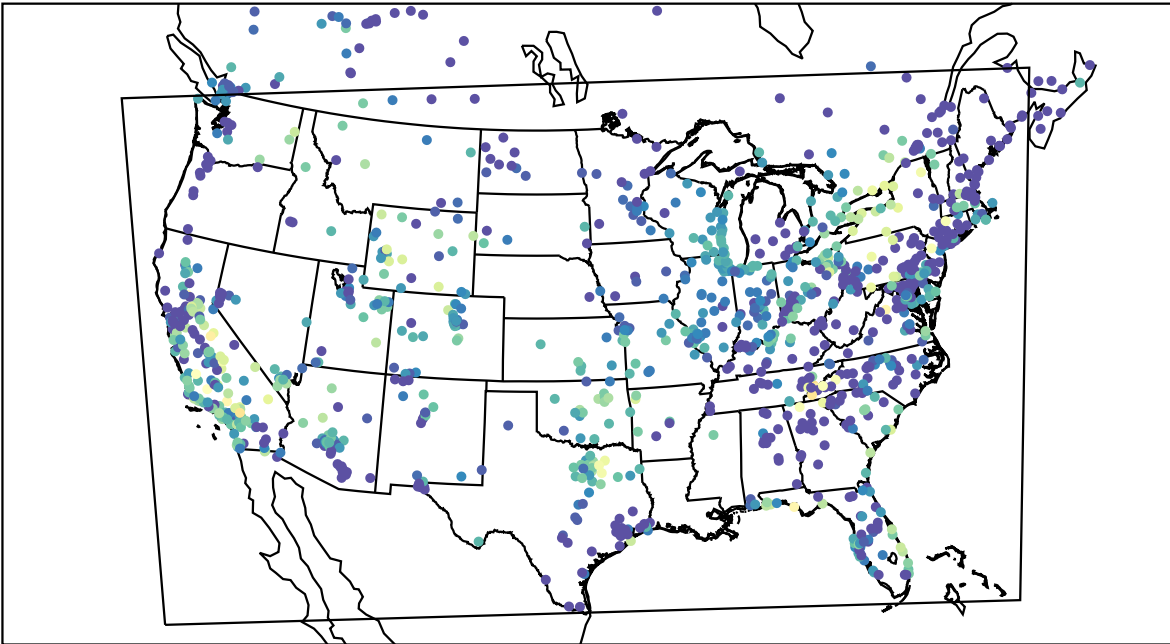
AirNOW (2019-09-26_07:00:00)
