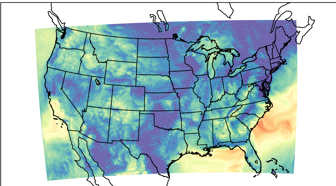
WRF (2019-09-25_11:00:00)
