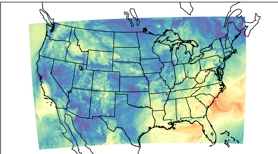
WRF (2019-09-25_15:00:00)
