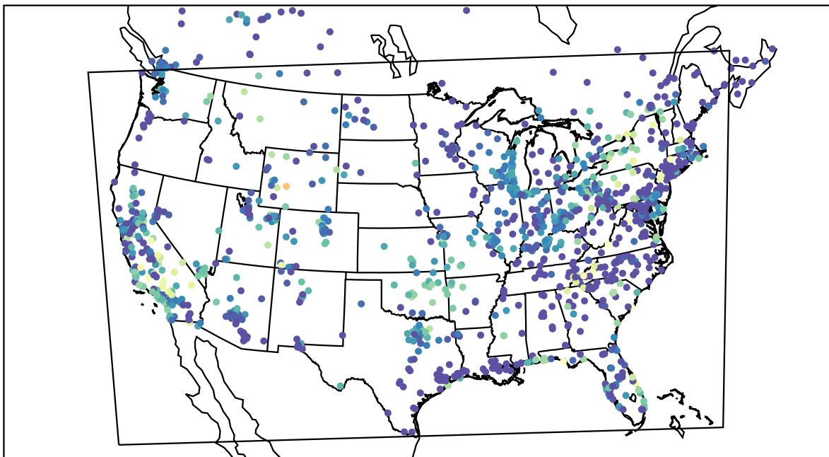
AirNOW (2019-09-26_09:00:00)
