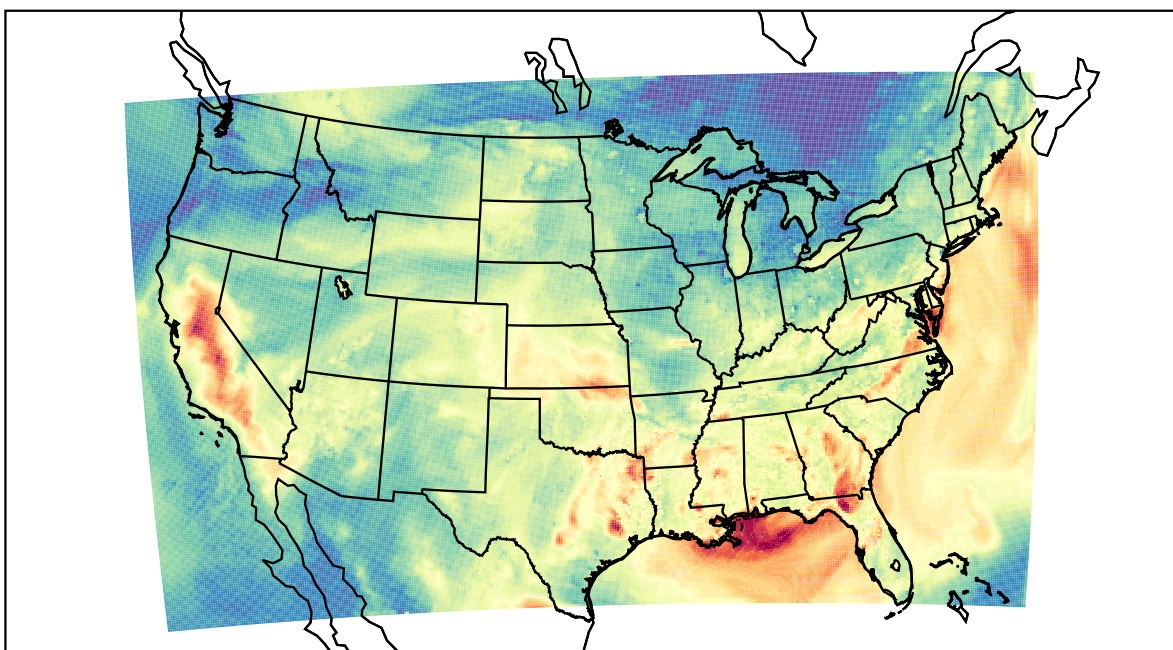
WRF (2019-09-26_23:00:00)
