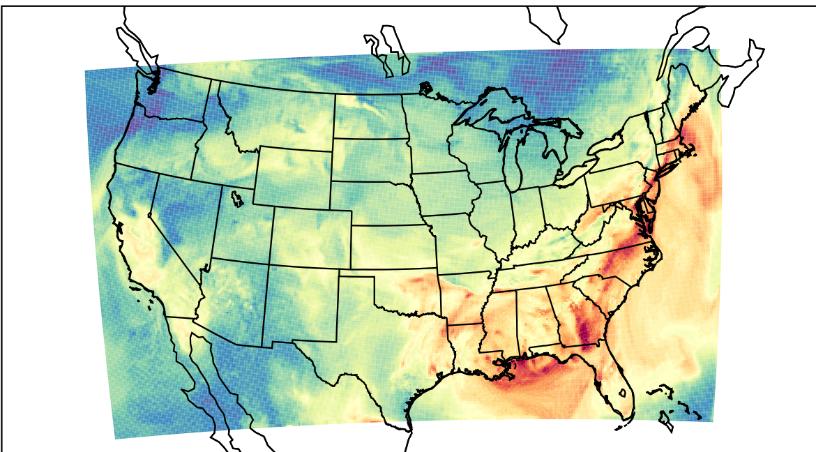
WRF (2019-09-26_18:00:00)
