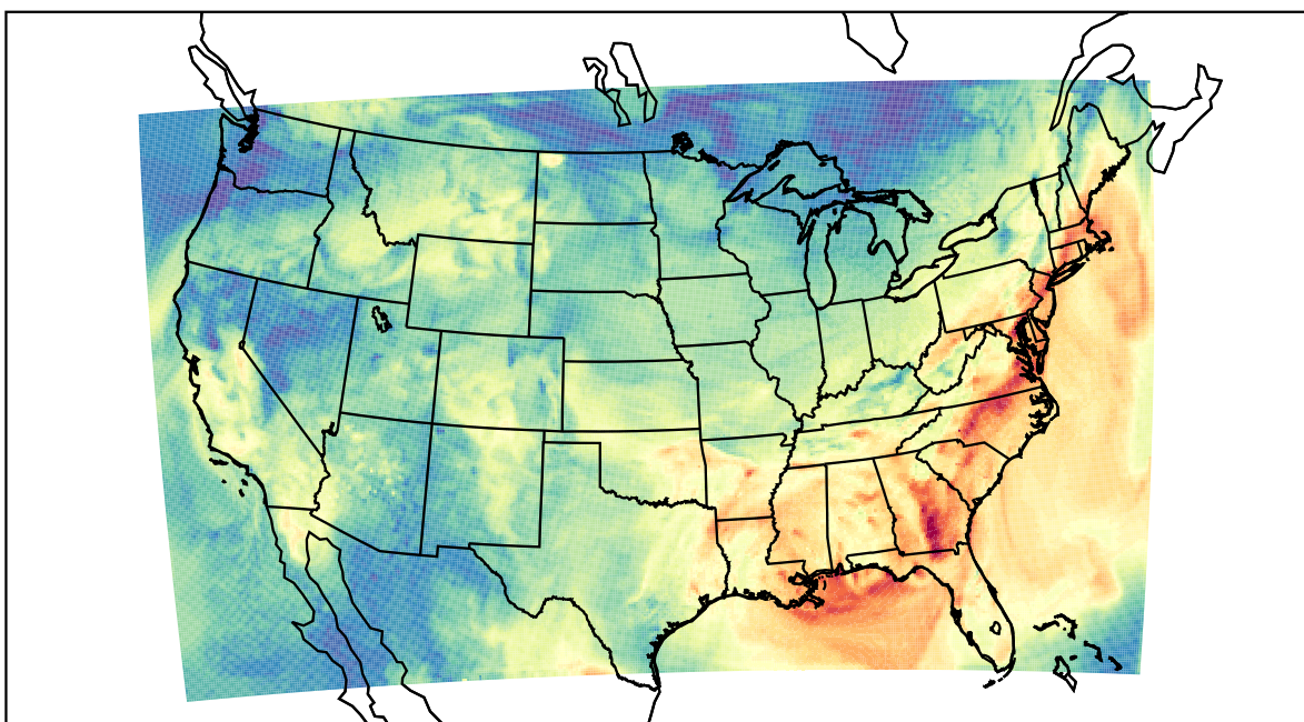
WRF (2019-09-26_17:00:00)
