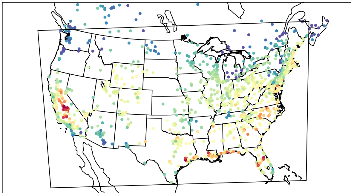
AirNOW (2019-09-26_20:00:00)
