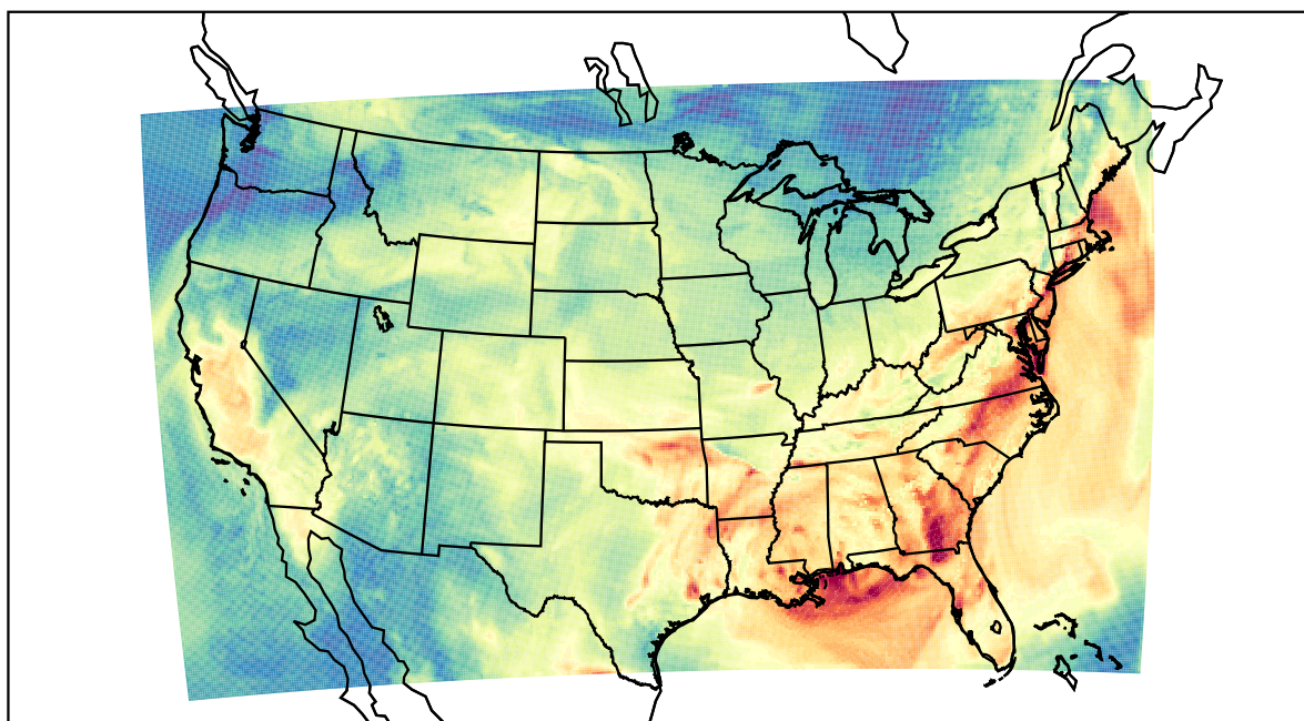
WRF (2019-09-26_19:00:00)
