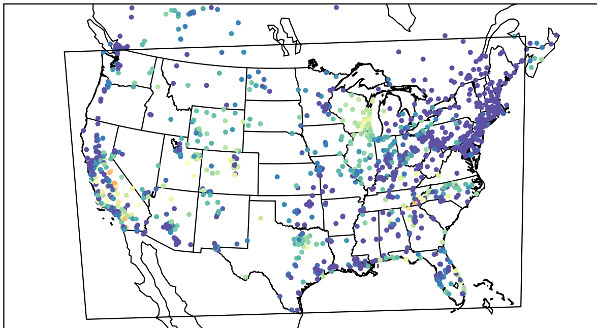
AirNOW (2019-09-25_04:00:00)
