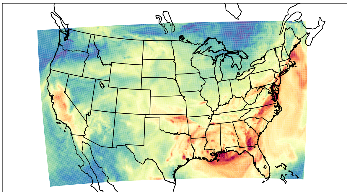
WRF (2019-09-26_20:00:00)
