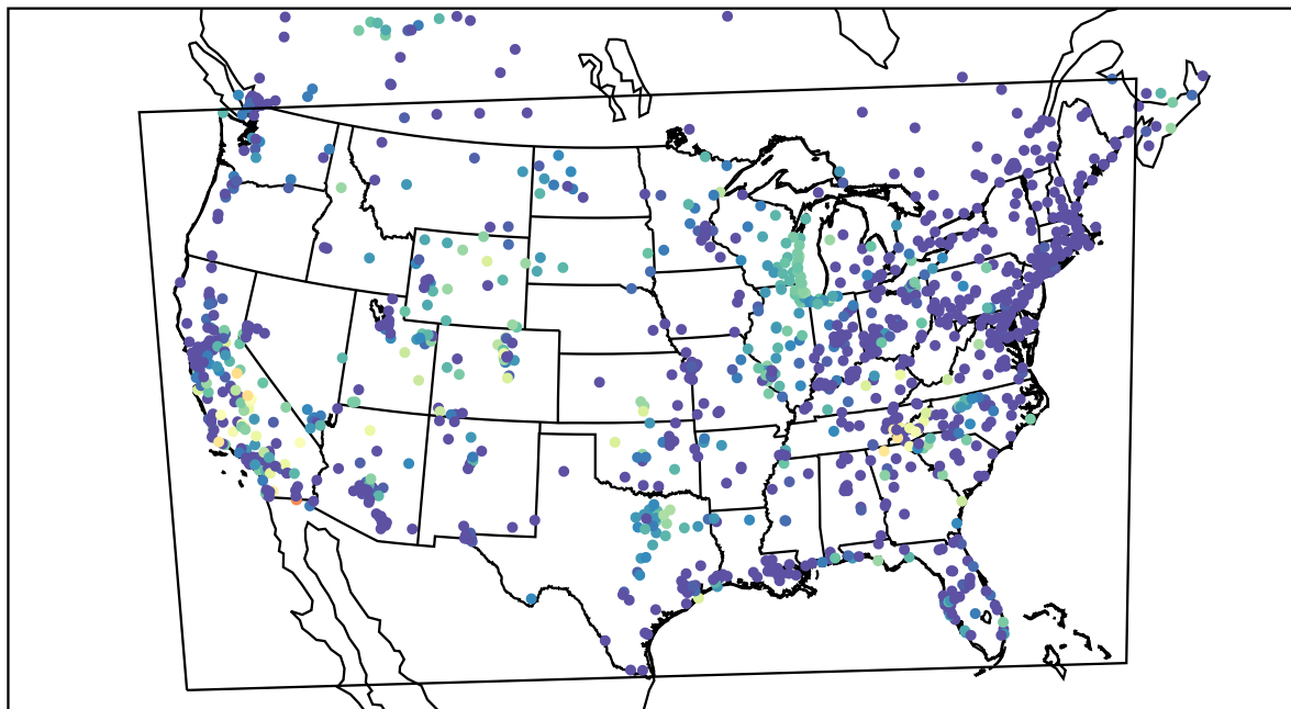
AirNOW (2019-09-25_09:00:00)
