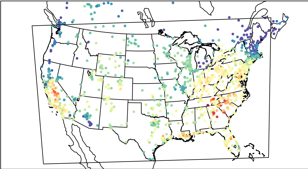
AirNOW (2019-09-25_18:00:00)
