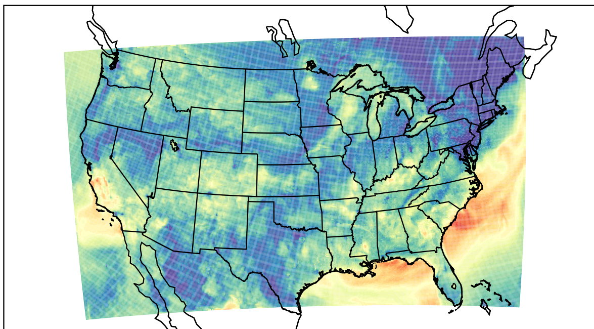
WRF (2019-09-25_05:00:00)
