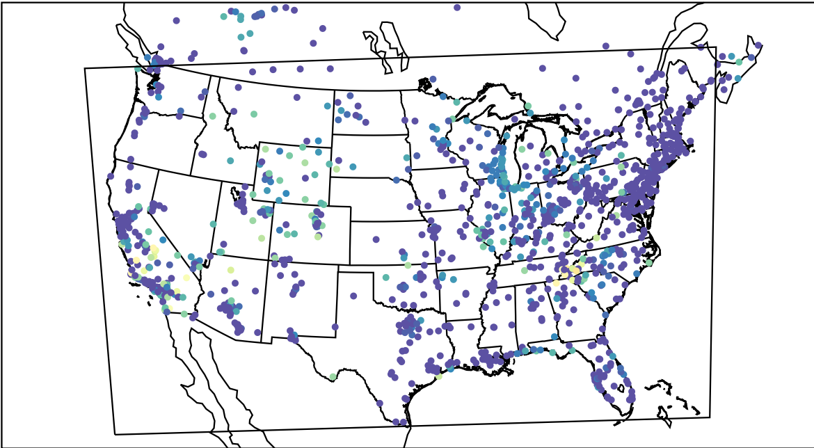
AirNOW (2019-09-25_12:00:00)
