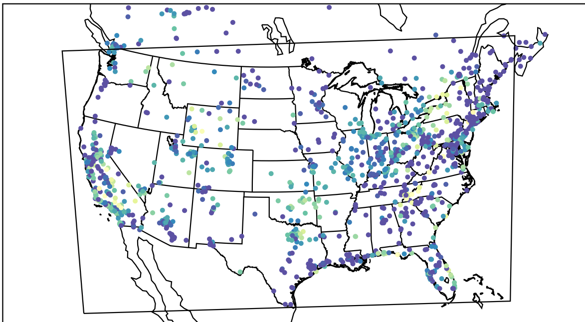
AirNOW (2019-09-26_08:00:00)
