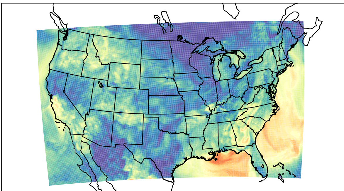
WRF (2019-09-26_08:00:00)
