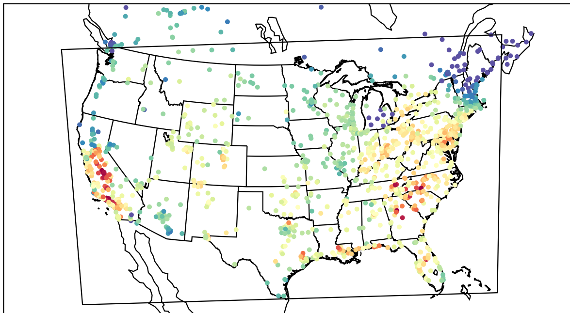
AirNOW (2019-09-25_20:00:00)
