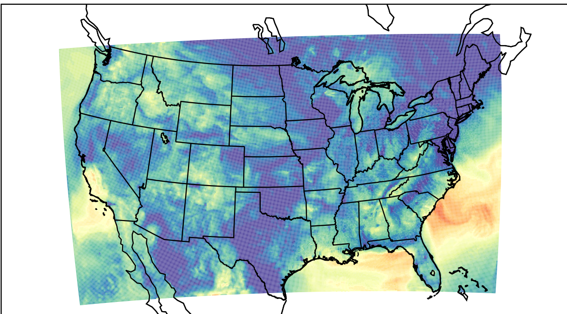
WRF (2019-09-25_12:00:00)
