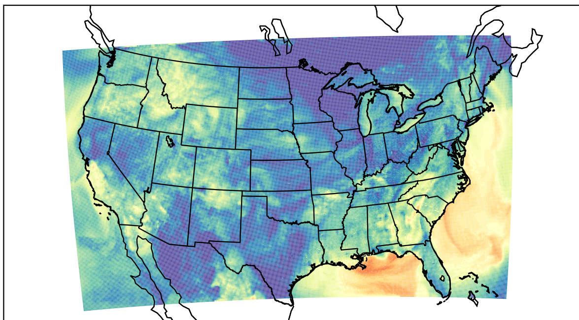
WRF (2019-09-26_10:00:00)
