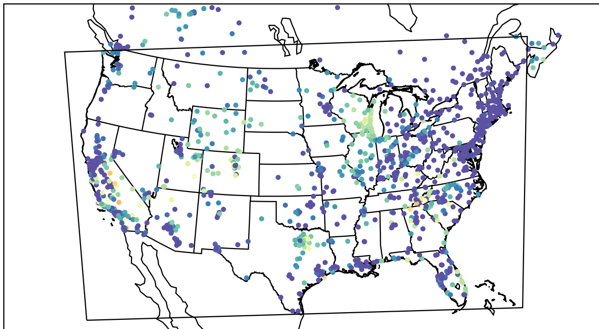
AirNOW (2019-09-25_06:00:00)
