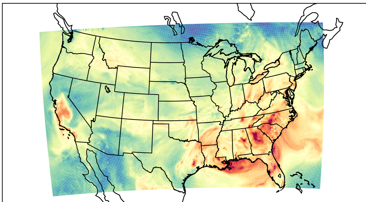
WRF (2019-09-25_20:00:00)
