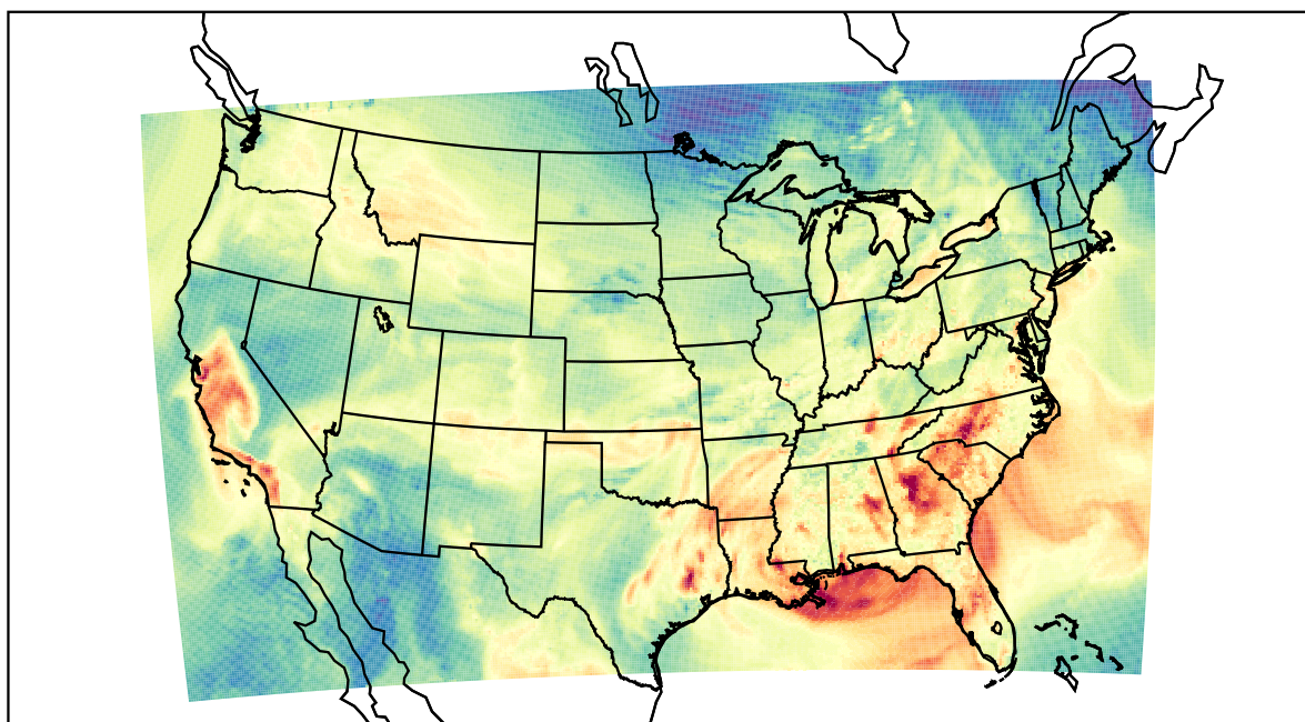
WRF (2019-09-25_22:00:00)
