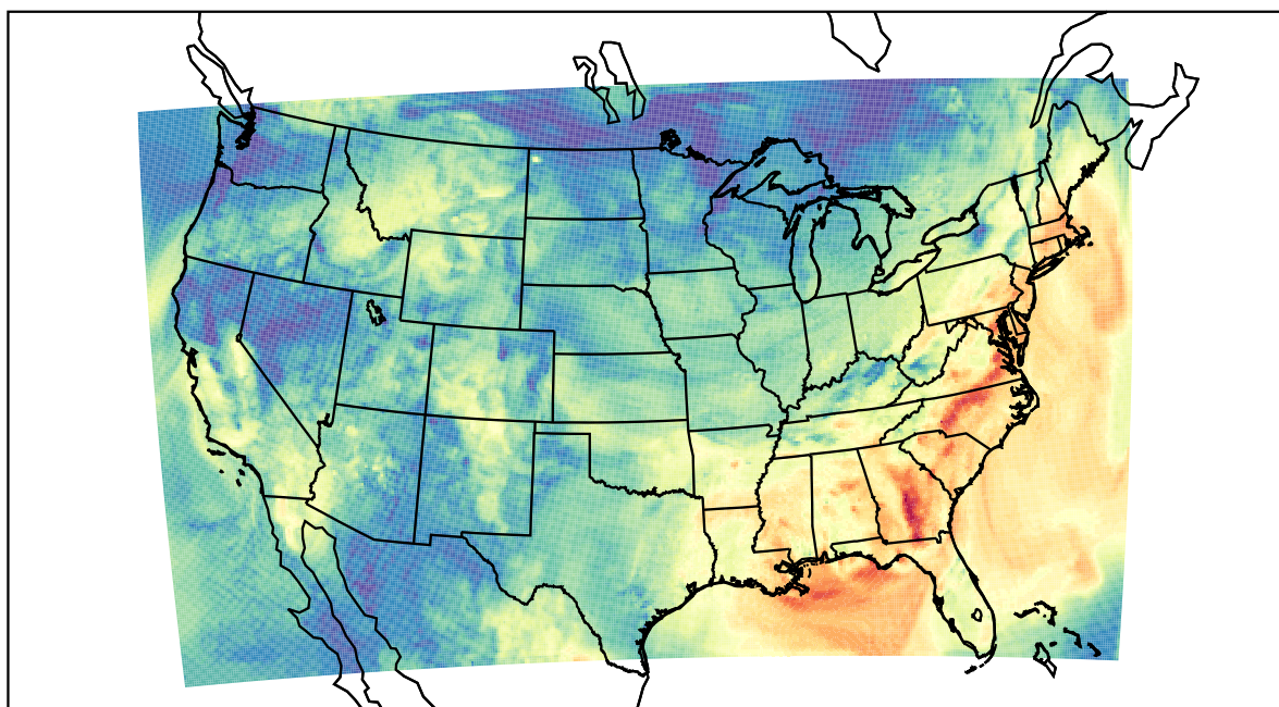
WRF (2019-09-26_16:00:00)
