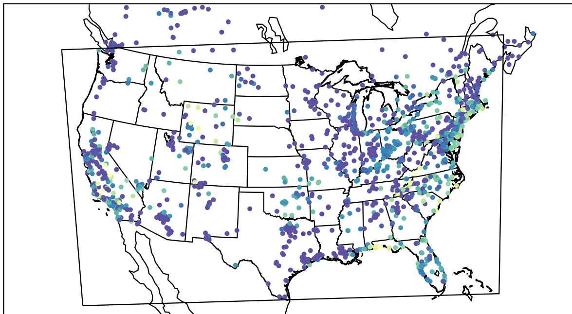
AirNOW (2019-09-26_13:00:00)
