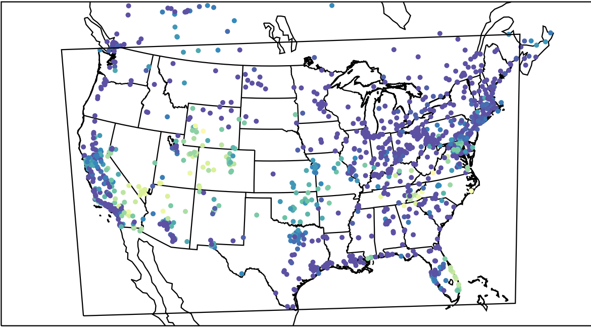
AirNOW (2019-09-30_08:00:00)
