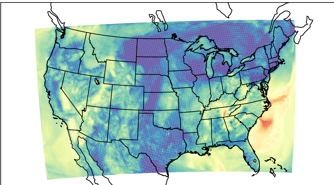
WRF (2019-09-30_10:00:00)
