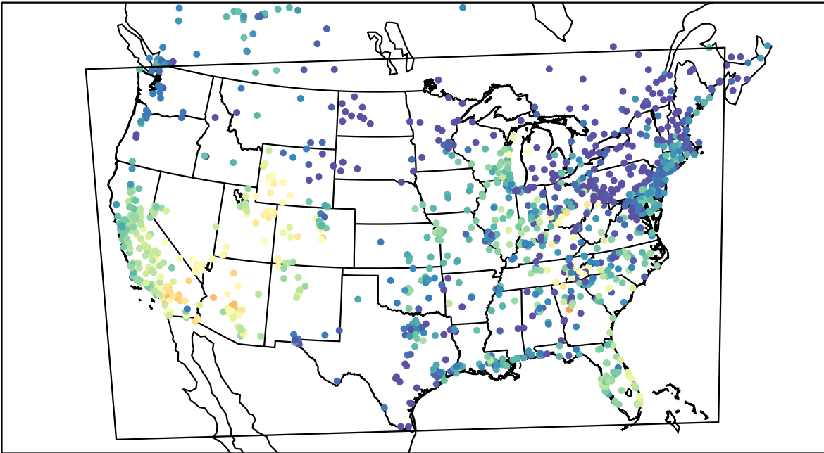
AirNOW (2019-10-01_00:00:00)
