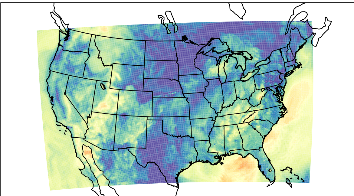
WRF (2019-10-01_11:00:00)
