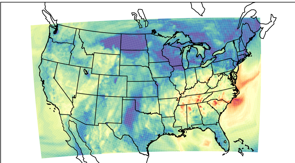
WRF (2019-09-30_02:00:00)
