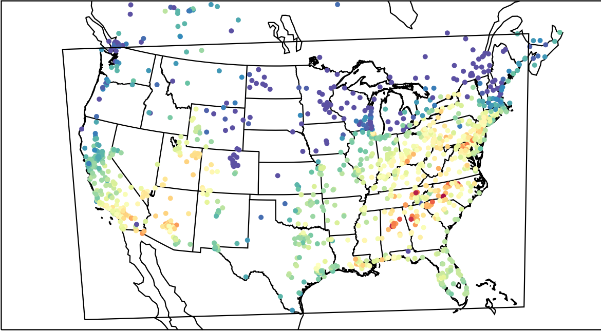
AirNOW (2019-10-01_20:00:00)
