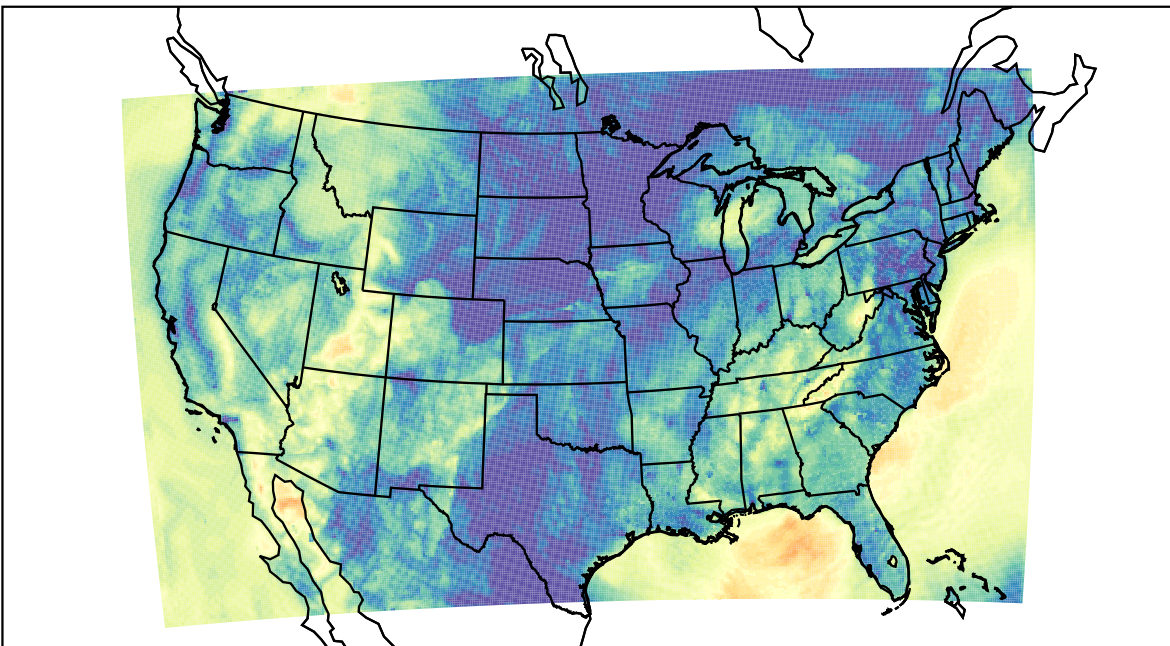
WRF (2019-10-01_12:00:00)
