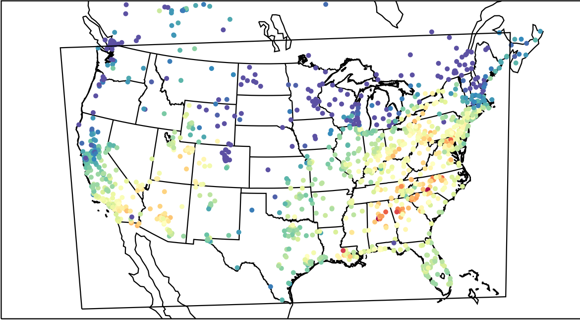
AirNOW (2019-10-01_19:00:00)
