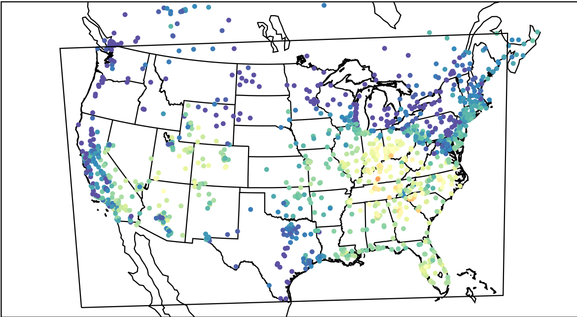
AirNOW (2019-09-30_16:00:00)
