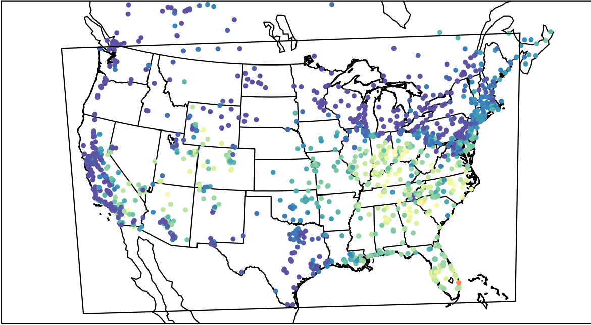
AirNOW (2019-09-30_15:00:00)
