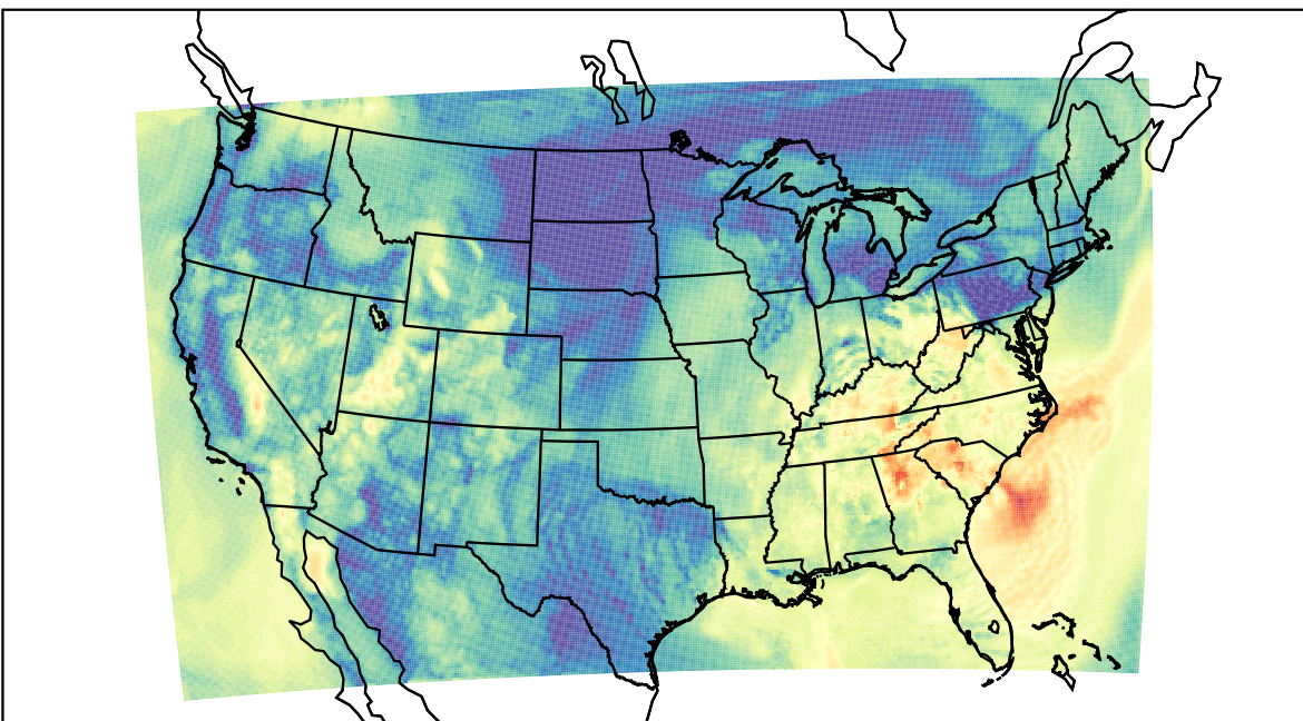
WRF (2019-09-30_15:00:00)
