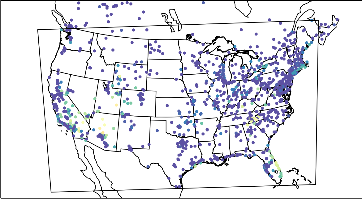
AirNOW (2019-10-01_11:00:00)
