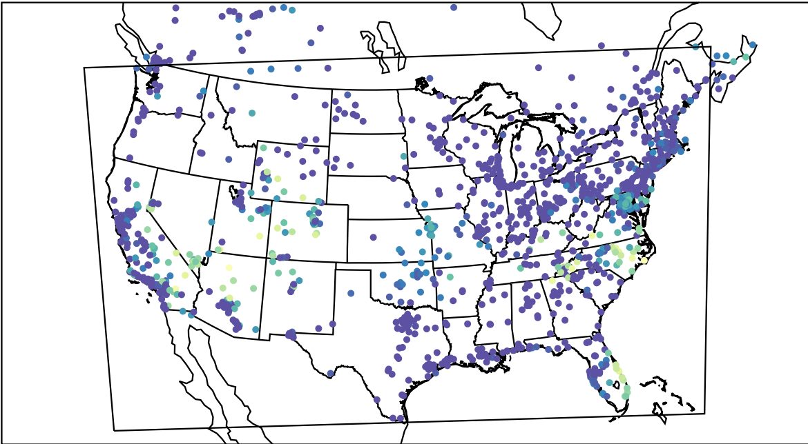
AirNOW (2019-09-30_12:00:00)
