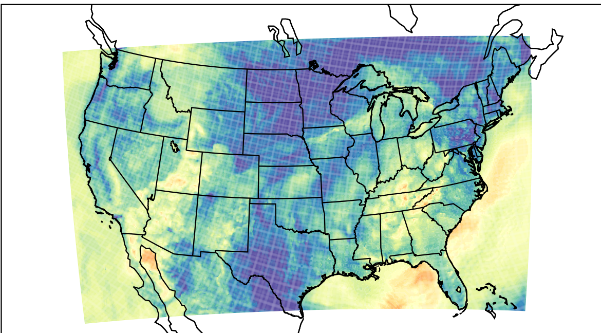
WRF (2019-10-01_08:00:00)
