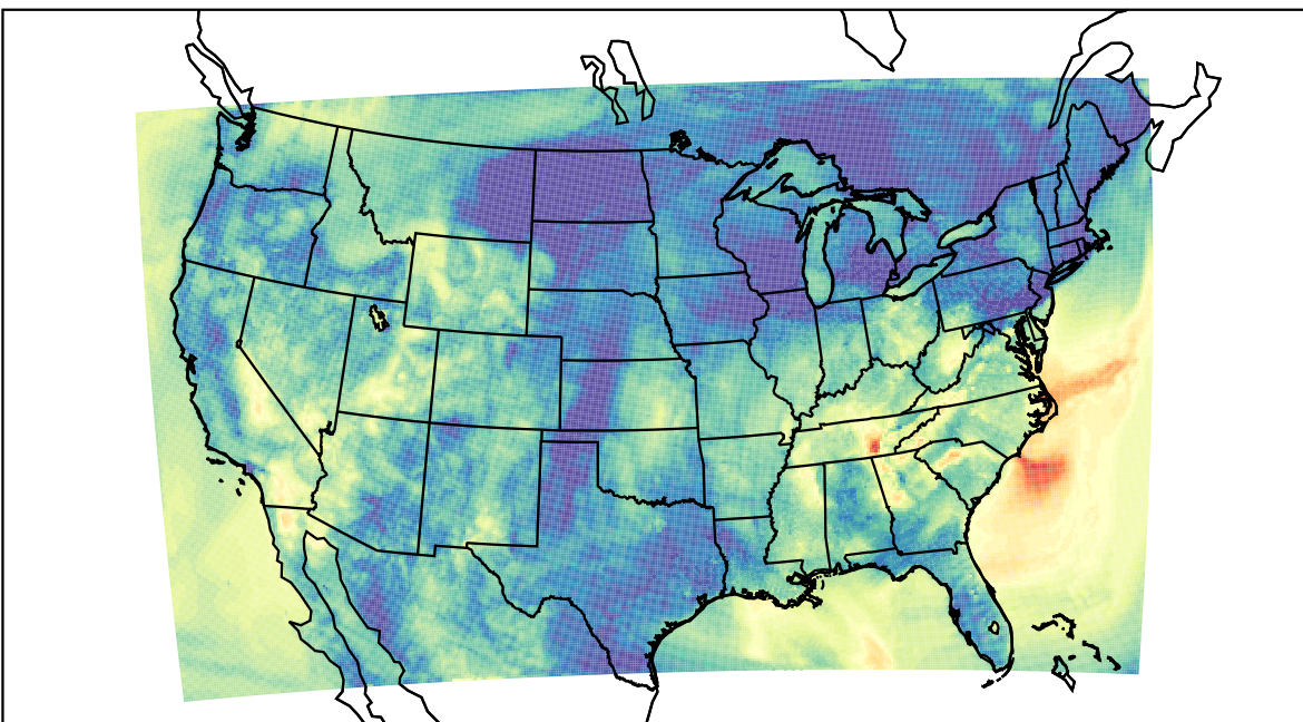
WRF (2019-09-30_08:00:00)
