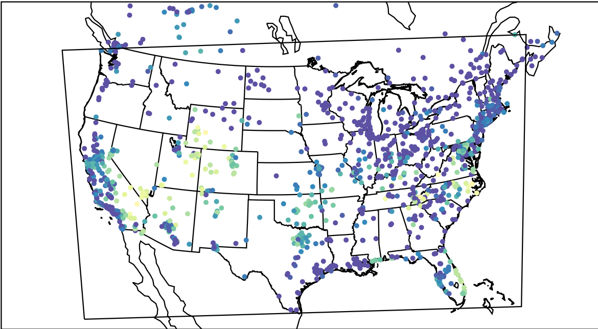
AirNOW (2019-09-30_06:00:00)
