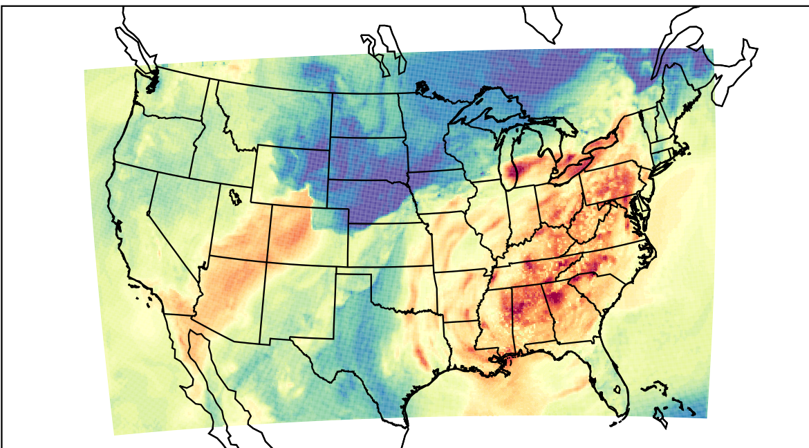
WRF (2019-10-01_21:00:00)
