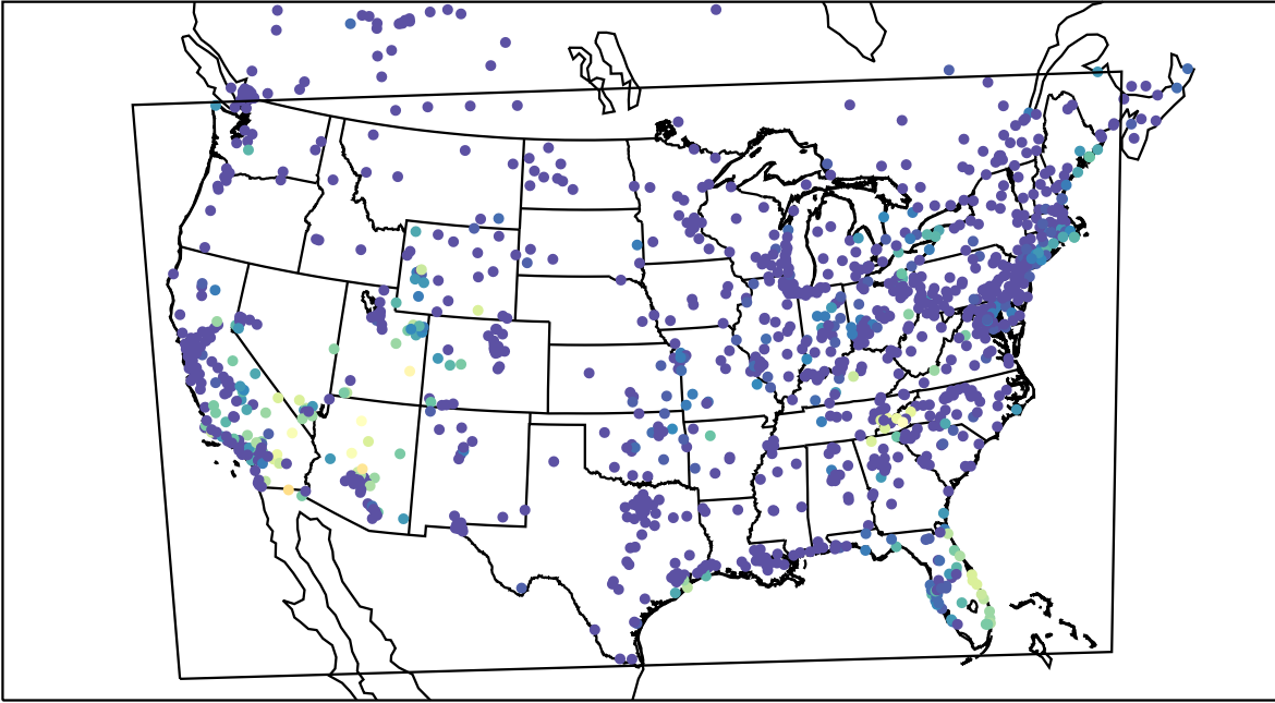
AirNOW (2019-10-01_12:00:00)
