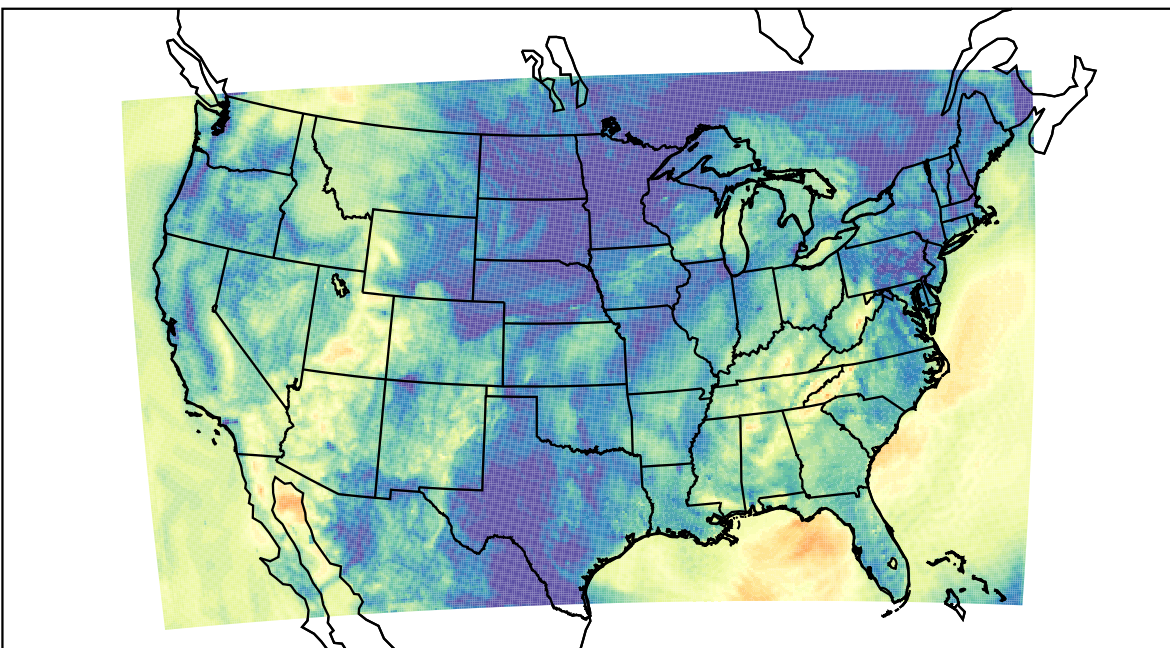
WRF (2019-10-01_10:00:00)
