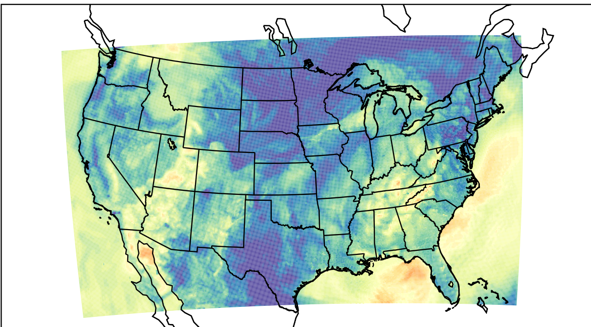
WRF (2019-10-01_09:00:00)
