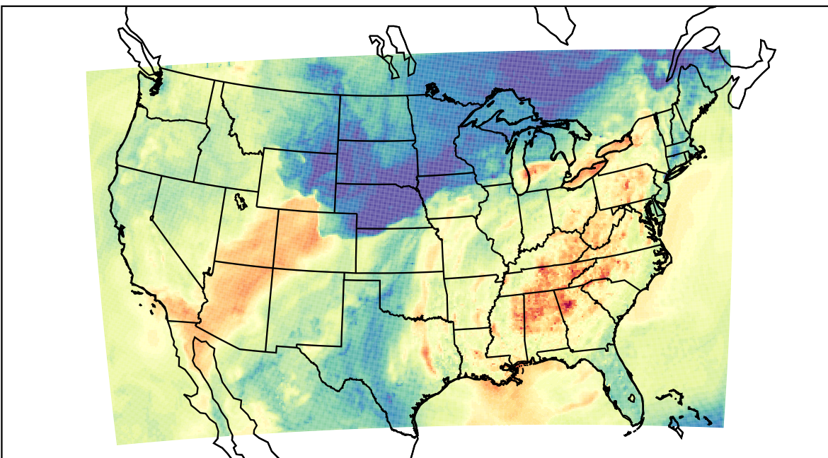
WRF (2019-10-01_23:00:00)
