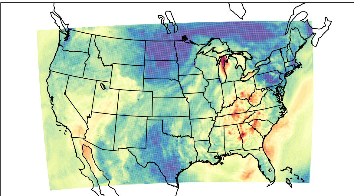
WRF (2019-10-01_01:00:00)
