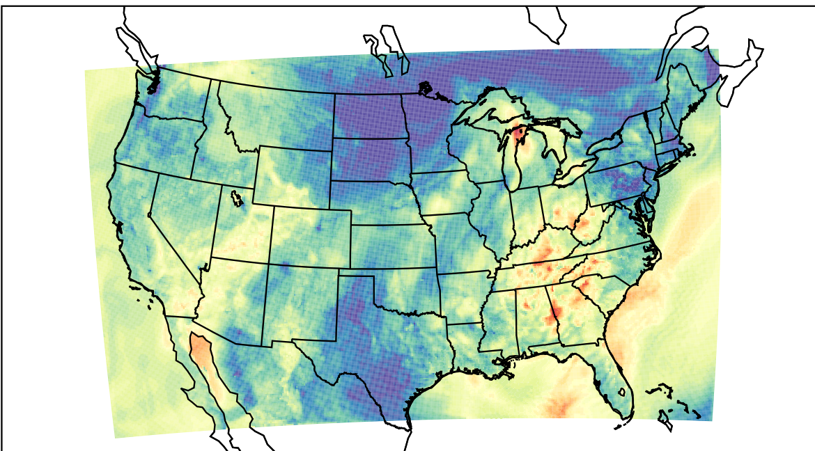
WRF (2019-10-01_03:00:00)
