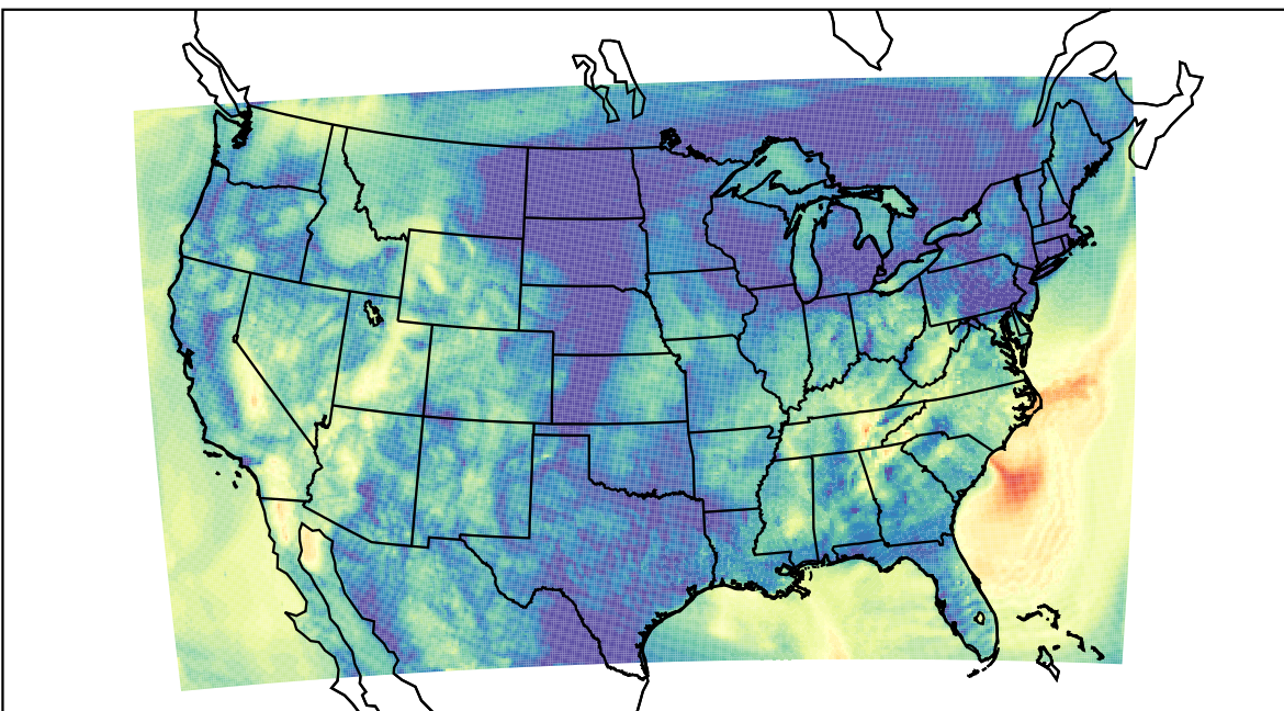
WRF (2019-09-30_12:00:00)
