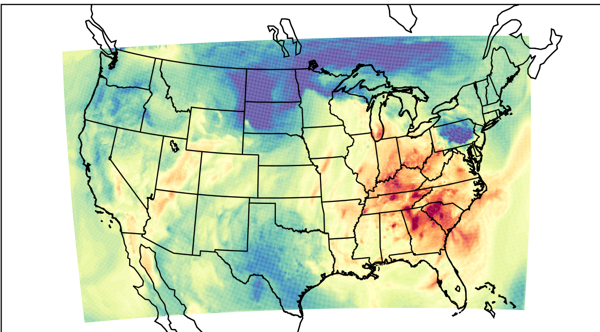
WRF (2019-09-30_18:00:00)
