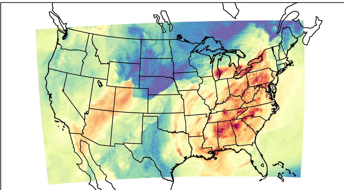
WRF (2019-10-01_20:00:00)
