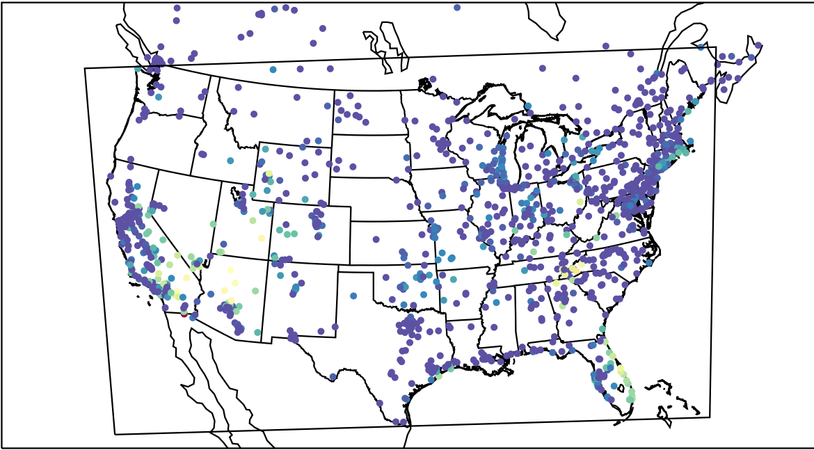
AirNOW (2019-10-01_10:00:00)
