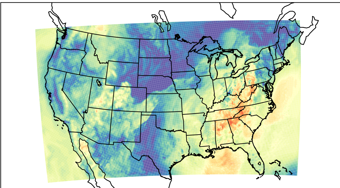
WRF (2019-10-01_15:00:00)
