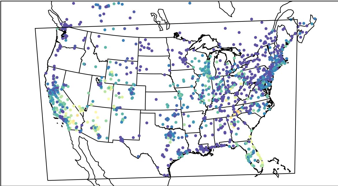
AirNOW (2019-10-01_04:00:00)
