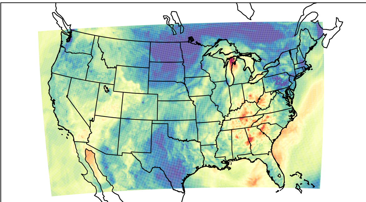
WRF (2019-10-01_02:00:00)
