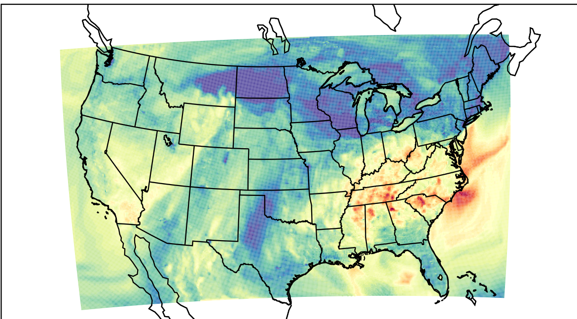
WRF (2019-09-30_01:00:00)
