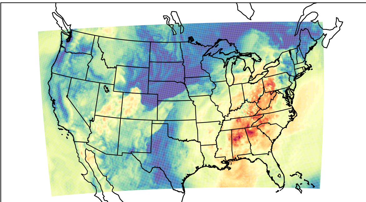
WRF (2019-10-01_16:00:00)
