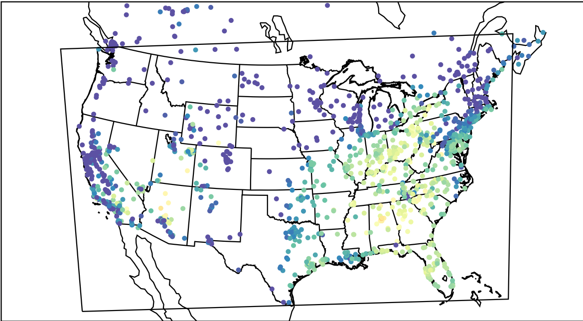
AirNOW (2019-10-01_15:00:00)
