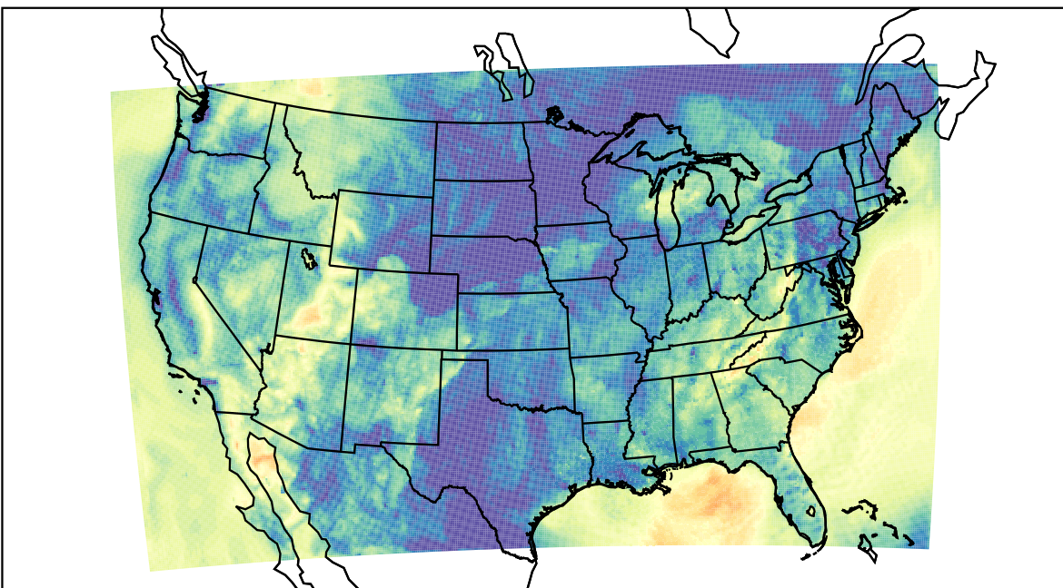
WRF (2019-10-01_13:00:00)
