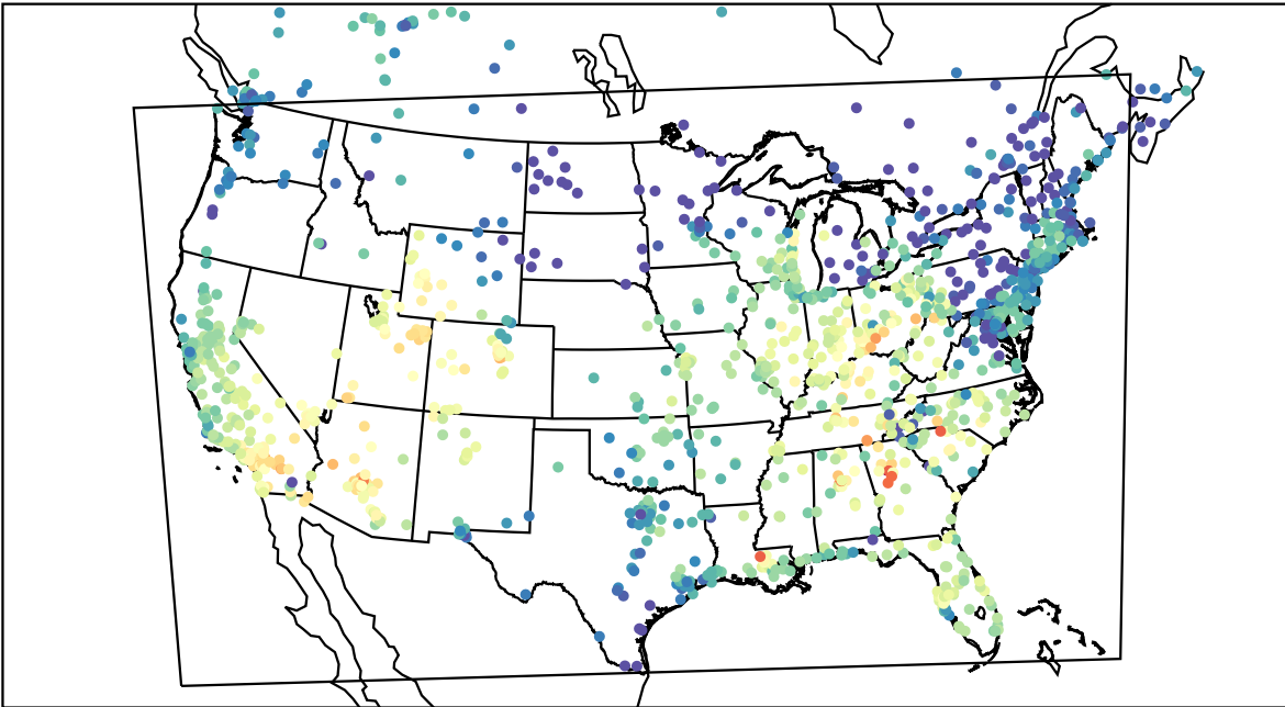
AirNOW (2019-09-30_22:00:00)
