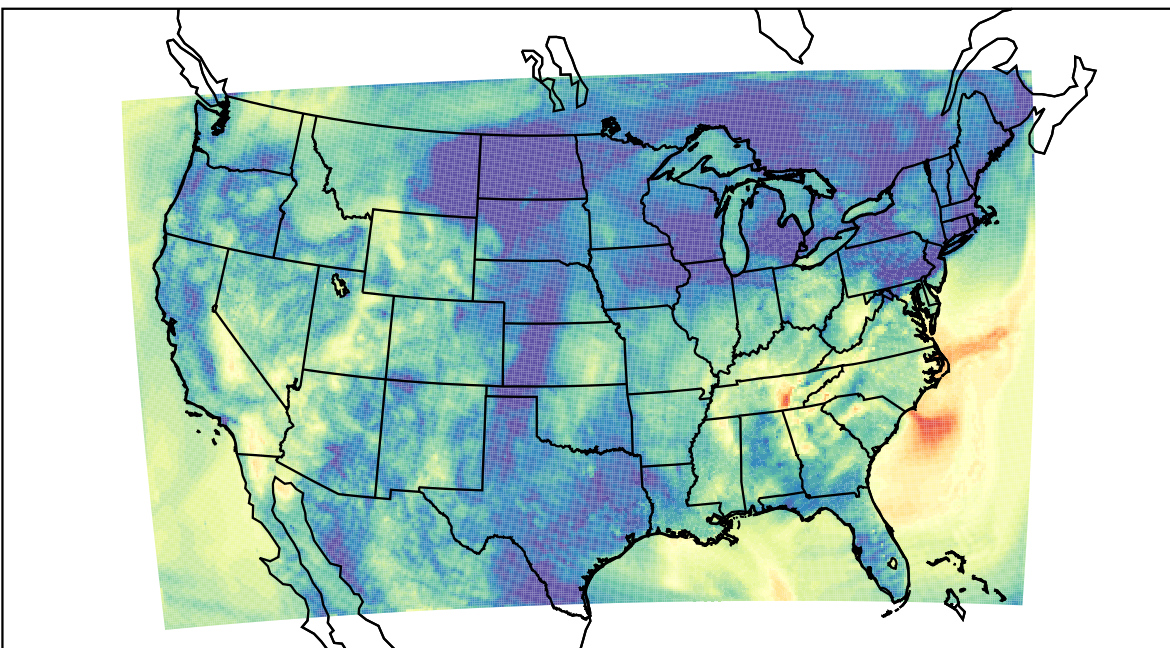
WRF (2019-09-30_09:00:00)
