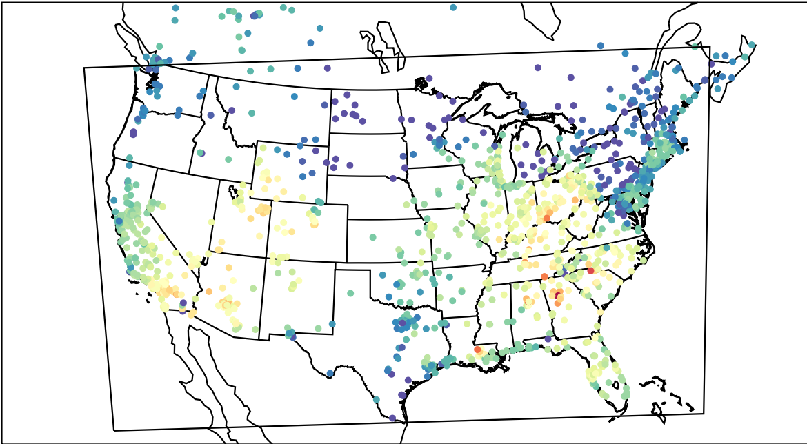
AirNOW (2019-09-30_21:00:00)
