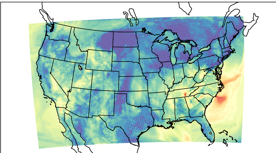
WRF (2019-09-30_07:00:00)
