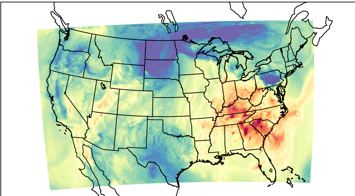
WRF (2019-09-30_17:00:00)
