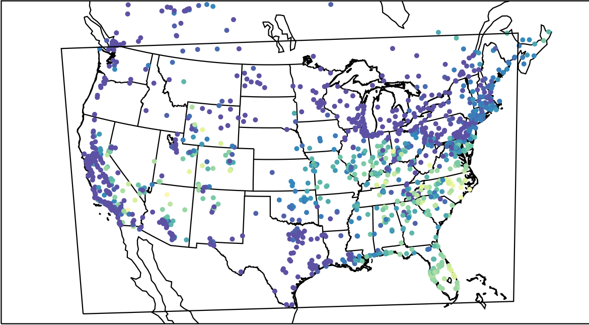
AirNOW (2019-09-30_14:00:00)
