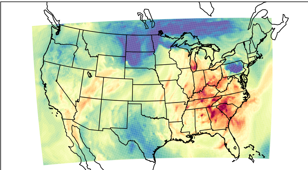
WRF (2019-09-30_19:00:00)
