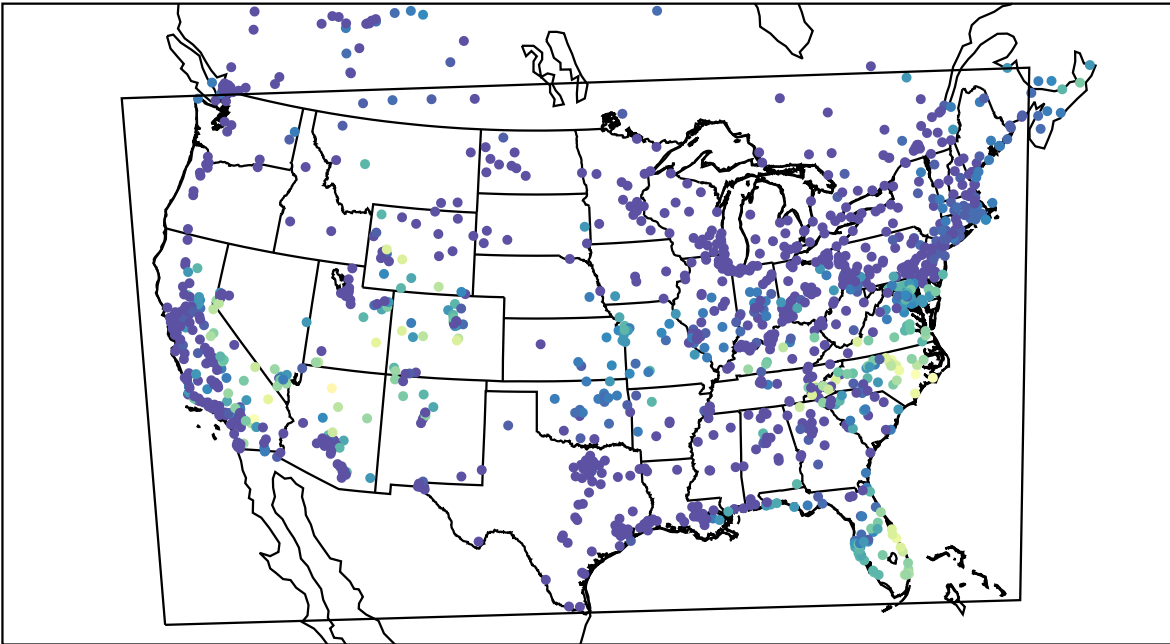
AirNOW (2019-09-30_13:00:00)
