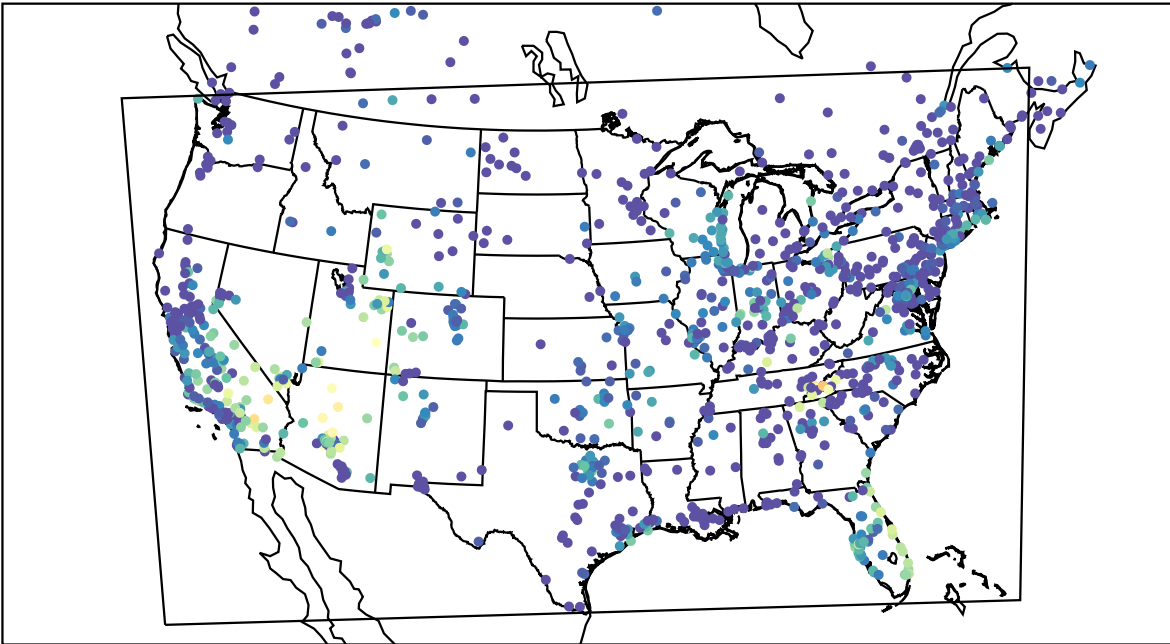
AirNOW (2019-10-01_07:00:00)
