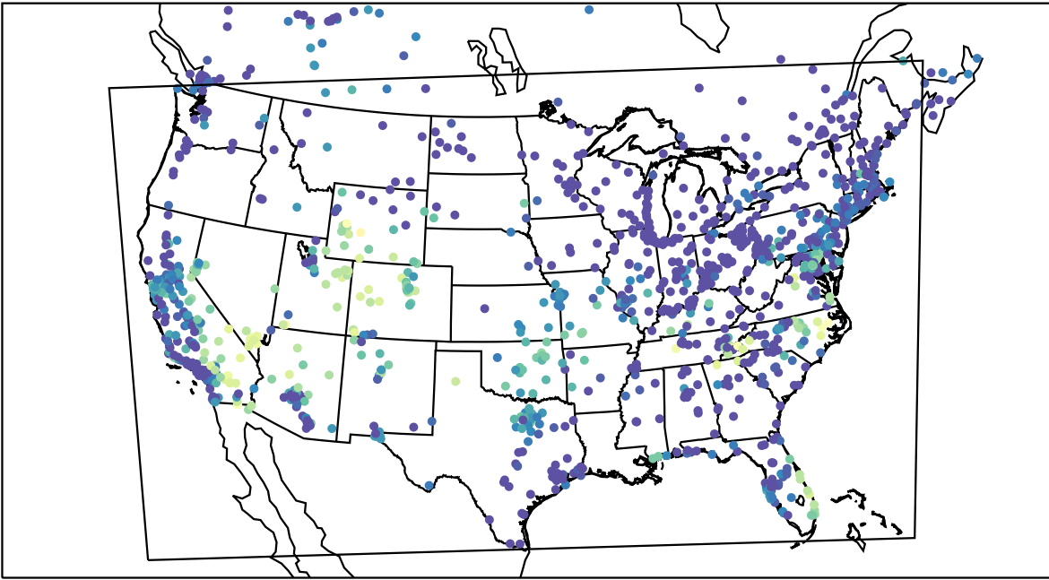
AirNOW (2019-09-30_07:00:00)
