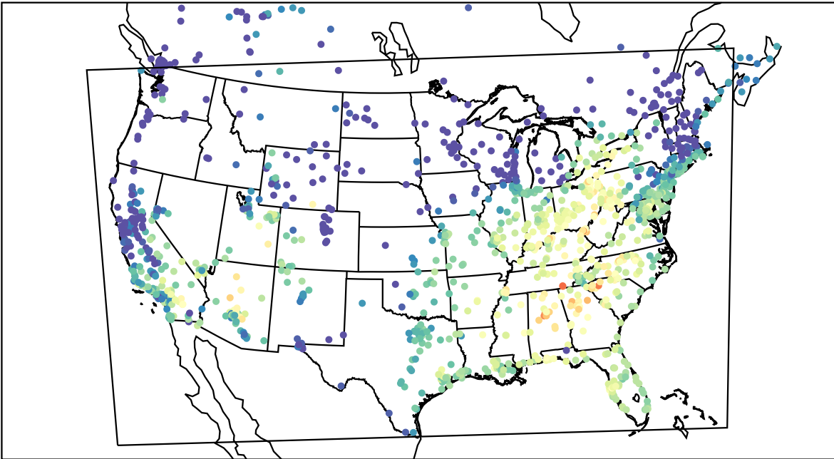
AirNOW (2019-10-01_16:00:00)
