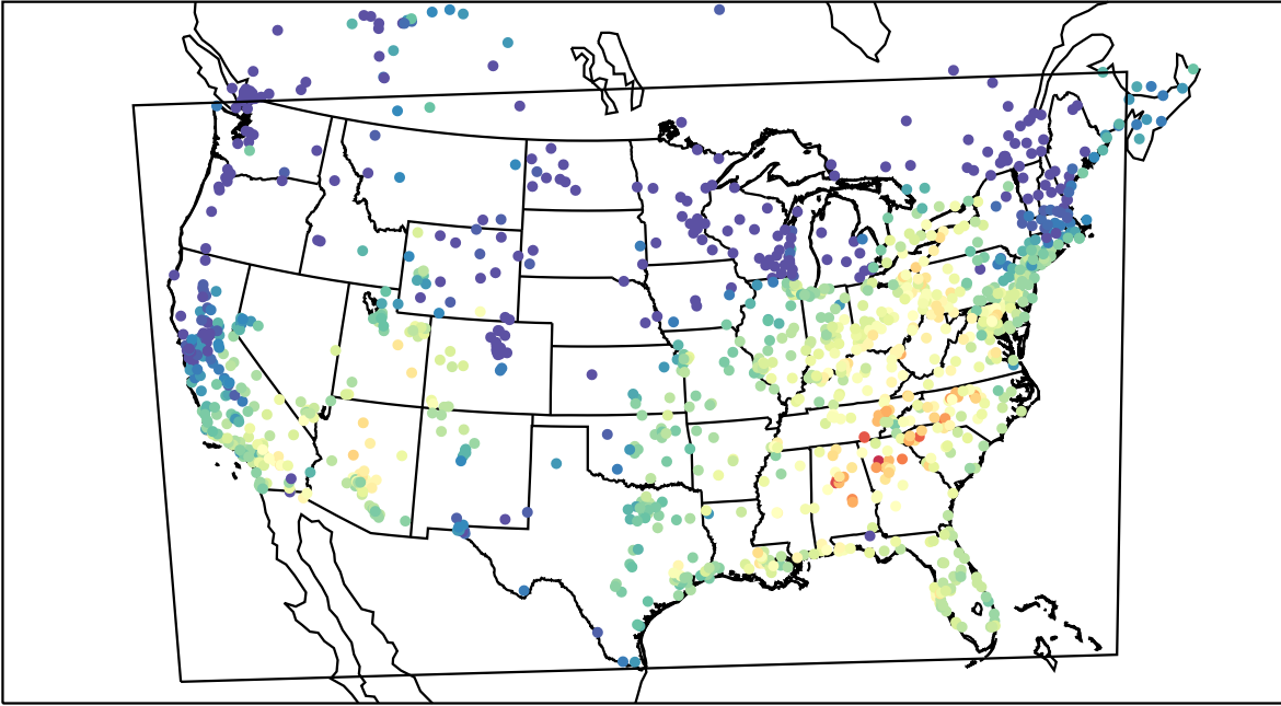
AirNOW (2019-10-01_17:00:00)
