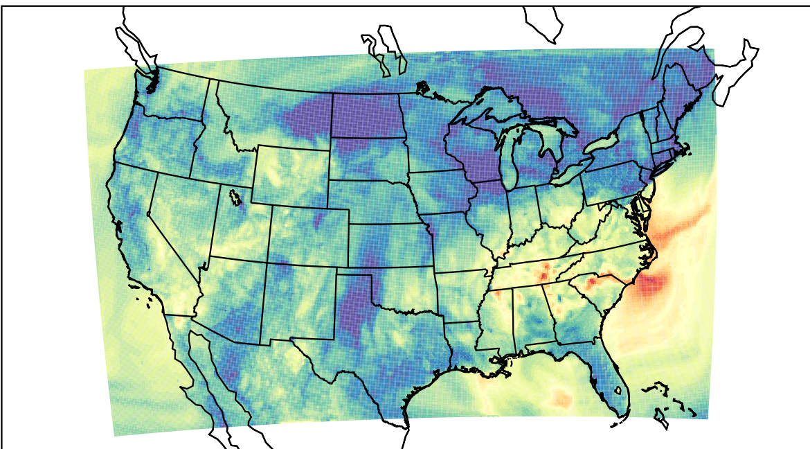
WRF (2019-09-30_04:00:00)
