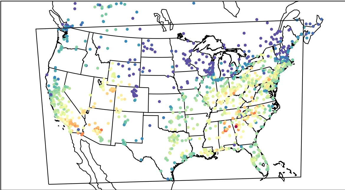
AirNOW (2019-10-01_22:00:00)
