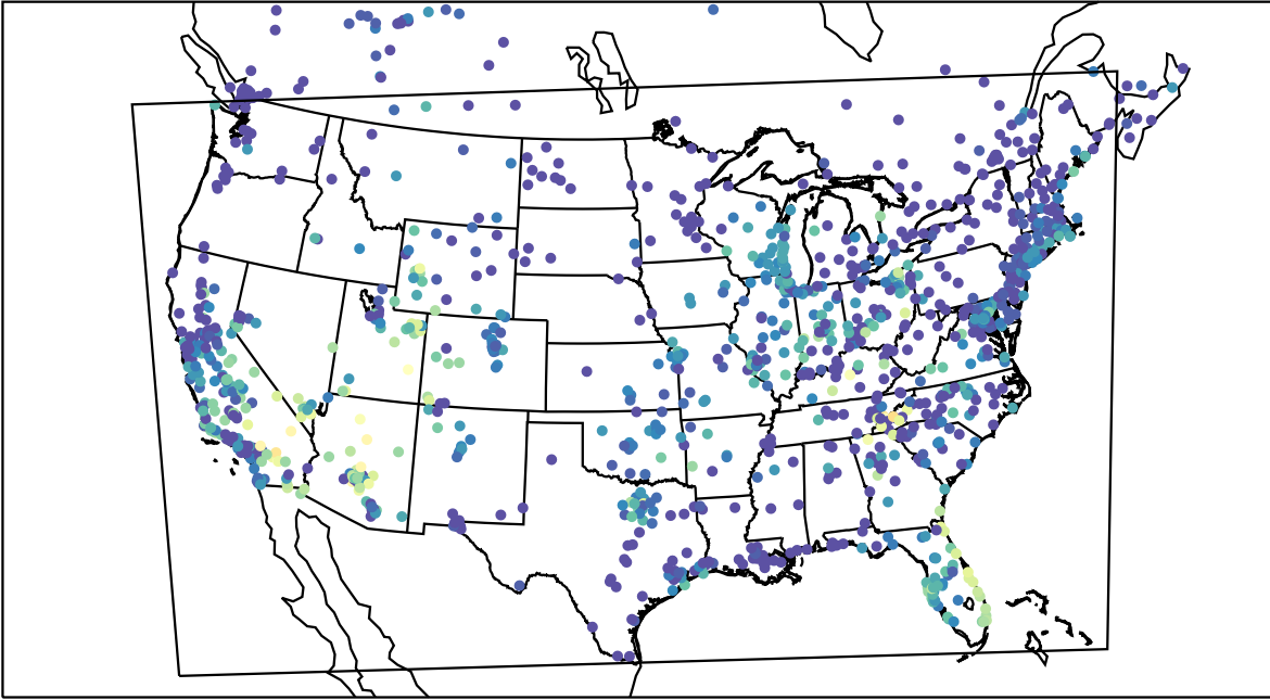
AirNOW (2019-10-01_06:00:00)
