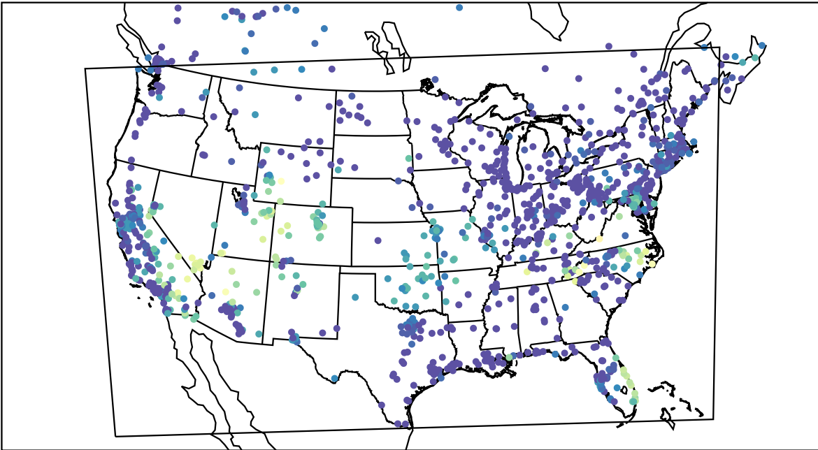
AirNOW (2019-09-30_09:00:00)
