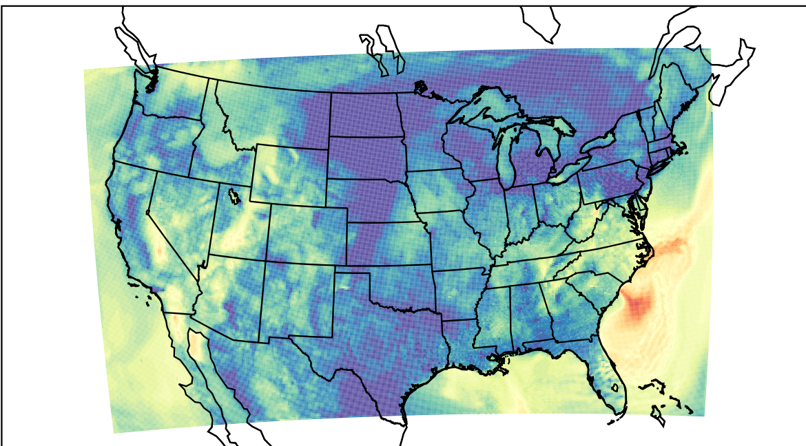
WRF (2019-09-30_13:00:00)
