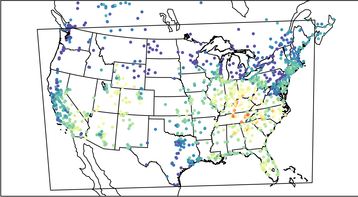
AirNOW (2019-09-30_17:00:00)
