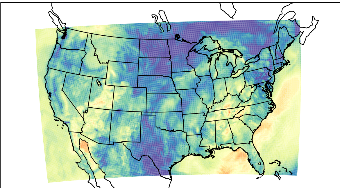
WRF (2019-10-01_07:00:00)
