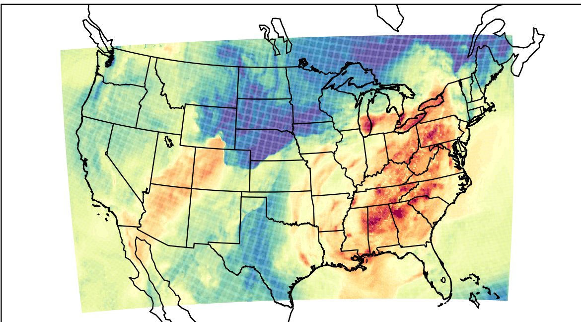
WRF (2019-10-01_19:00:00)
