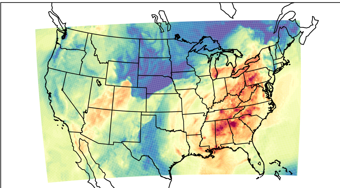
WRF (2019-10-01_18:00:00)
