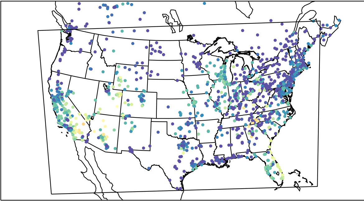
AirNOW (2019-10-01_03:00:00)
