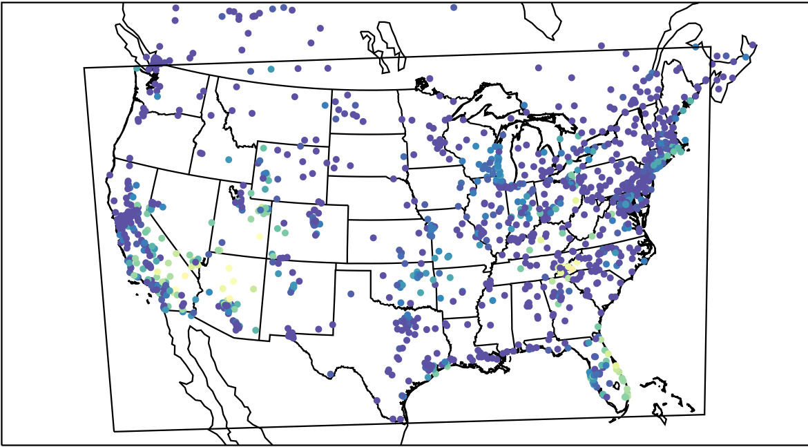
AirNOW (2019-10-01_09:00:00)
