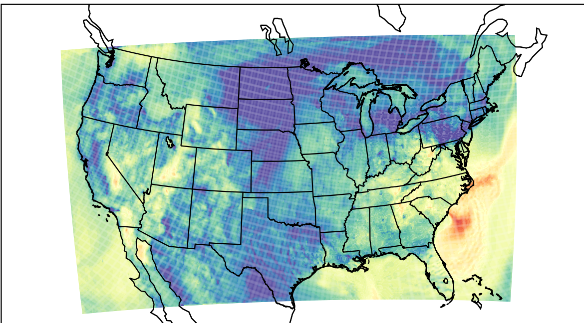
WRF (2019-09-30_14:00:00)
