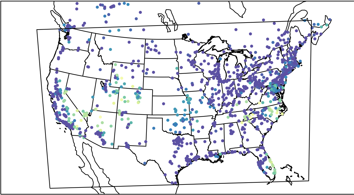
AirNOW (2019-09-30_11:00:00)
