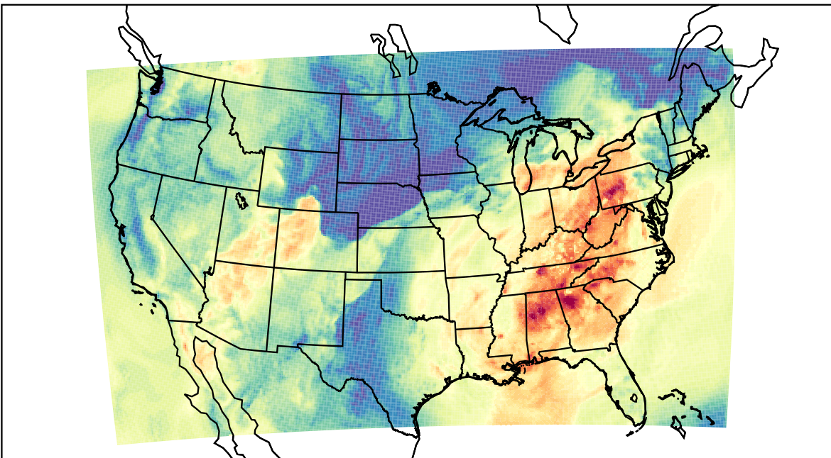
WRF (2019-10-01_17:00:00)
