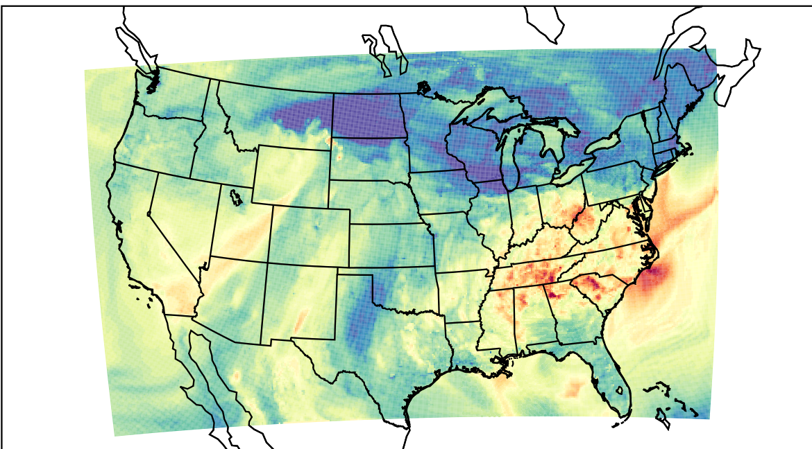
WRF (2019-09-30_00:00:00)
