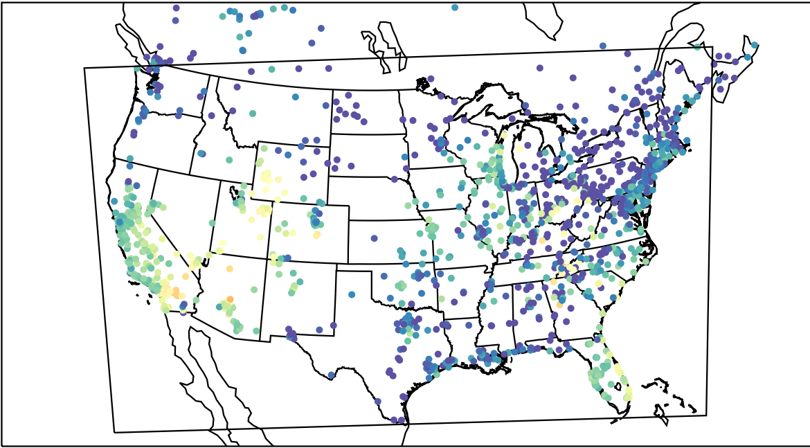
AirNOW (2019-10-01_01:00:00)
