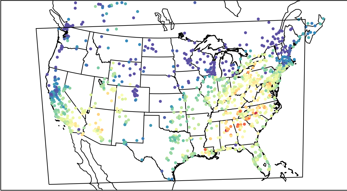
AirNOW (2019-10-01_18:00:00)
