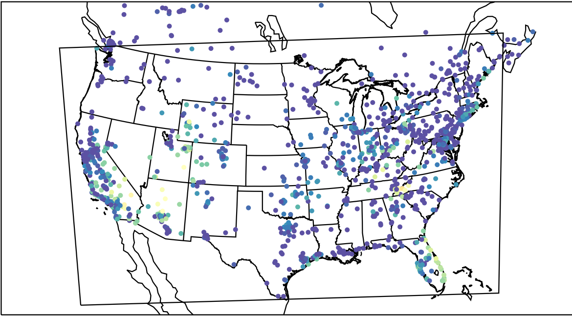
AirNOW (2019-10-01_08:00:00)
