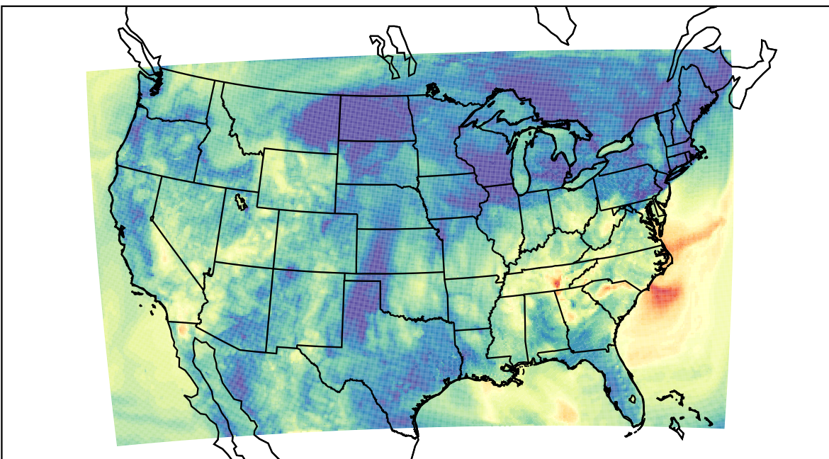
WRF (2019-09-30_06:00:00)
