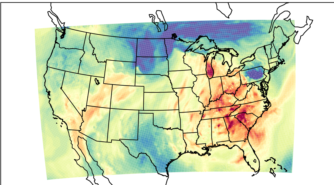
WRF (2019-09-30_20:00:00)
