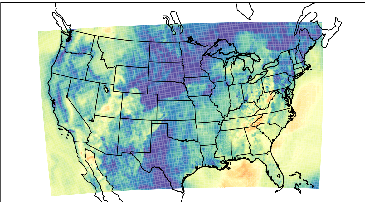
WRF (2019-10-01_14:00:00)
