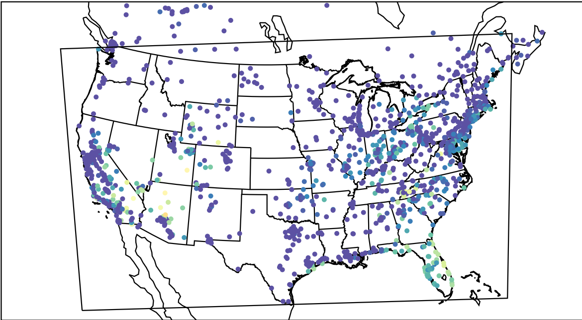
AirNOW (2019-10-01_13:00:00)
