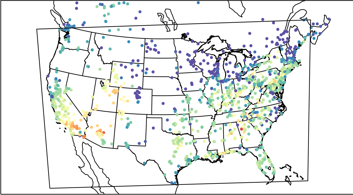
AirNOW (2019-10-01_23:00:00)
