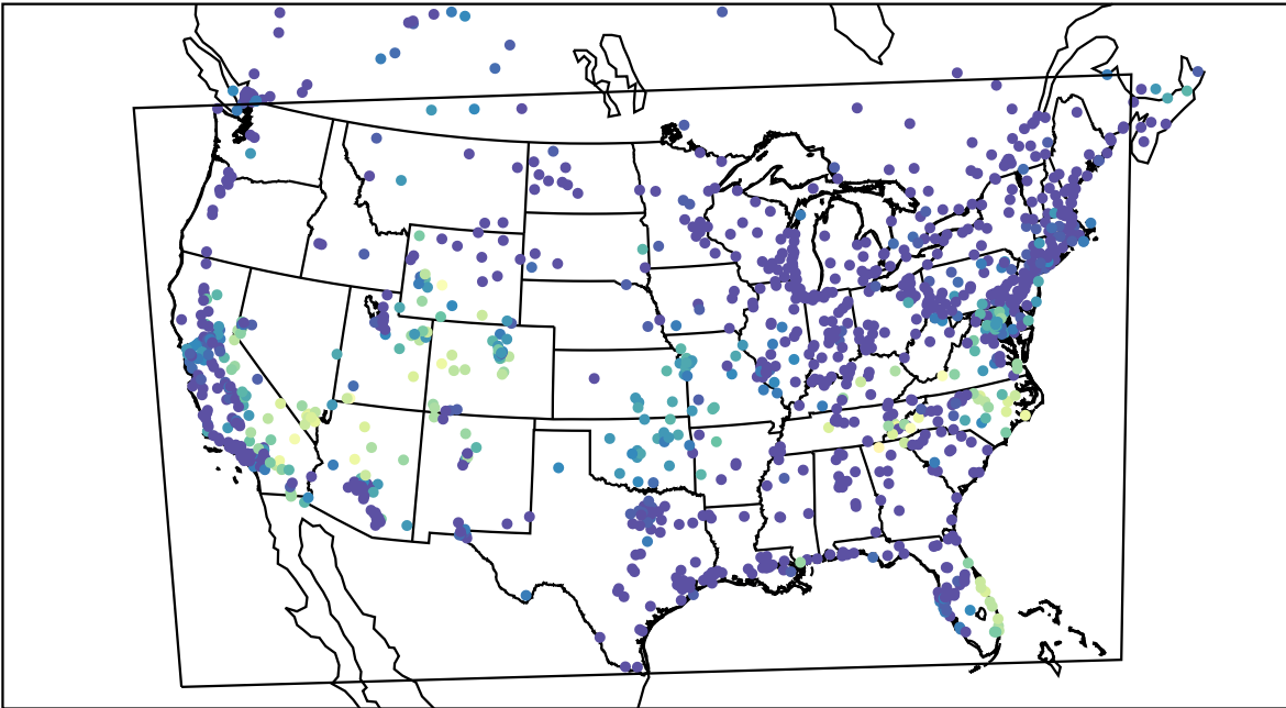
AirNOW (2019-09-30_10:00:00)
