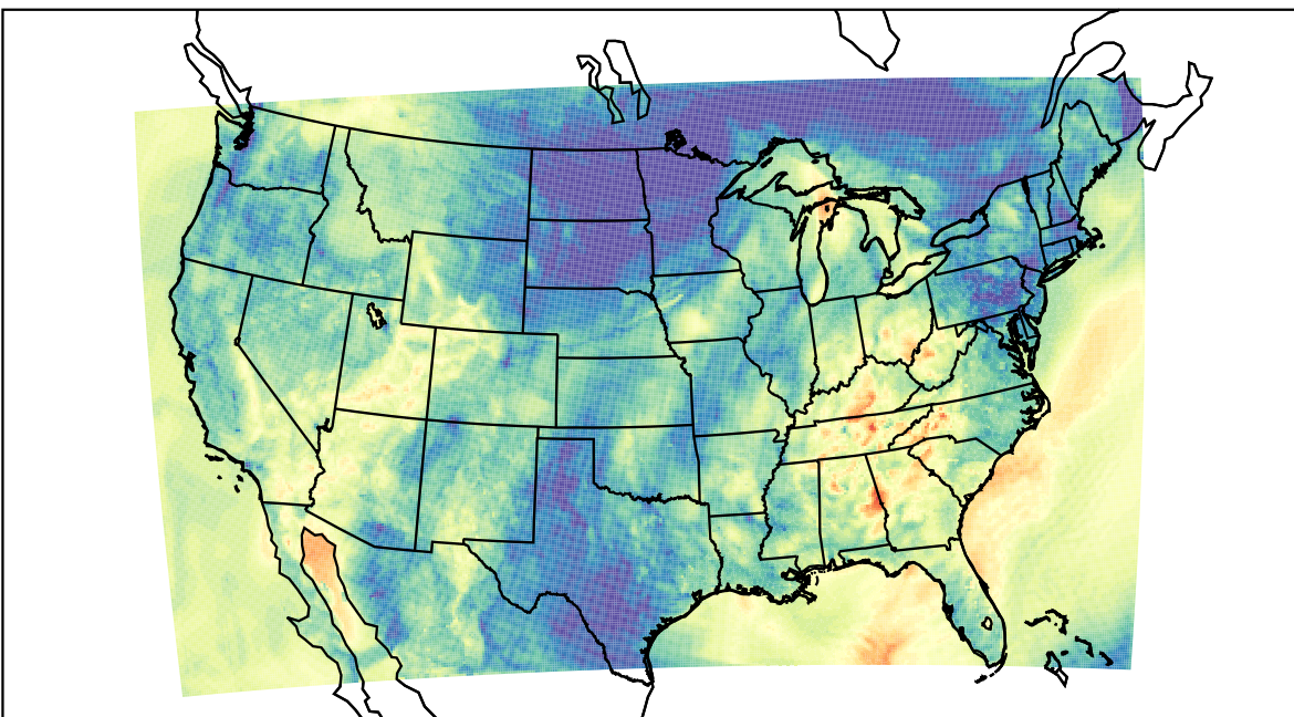
WRF (2019-10-01_04:00:00)
