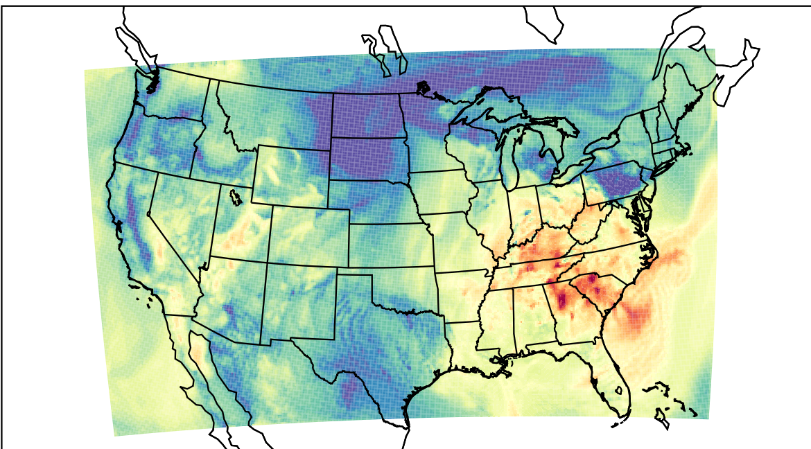
WRF (2019-09-30_16:00:00)
