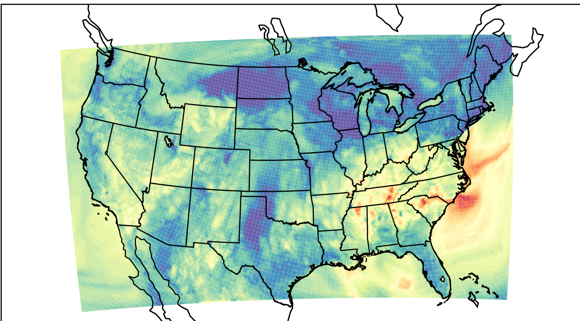
WRF (2019-09-30_03:00:00)
