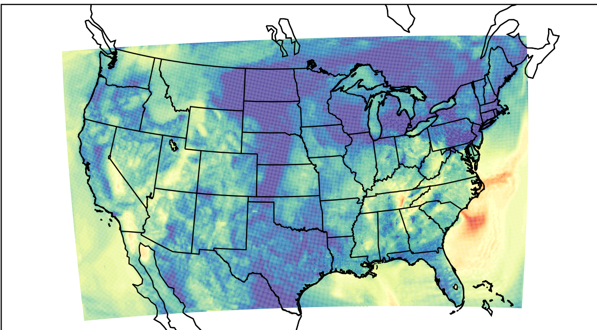
WRF (2019-09-30_11:00:00)
