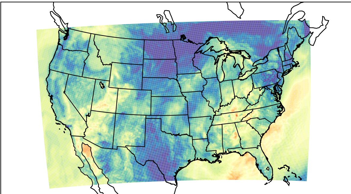
WRF (2019-10-01_06:00:00)
