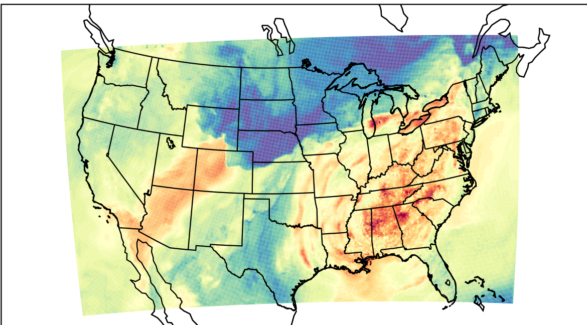
WRF (2019-10-01_22:00:00)
