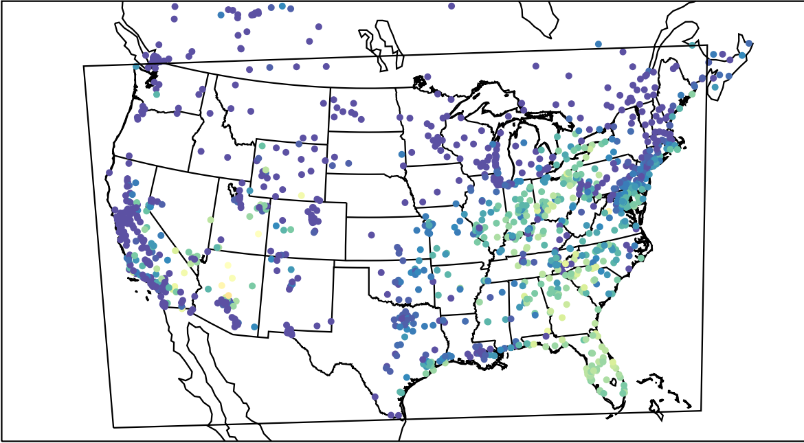
AirNOW (2019-10-01_14:00:00)
