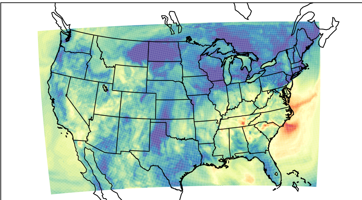
WRF (2019-09-30_05:00:00)
