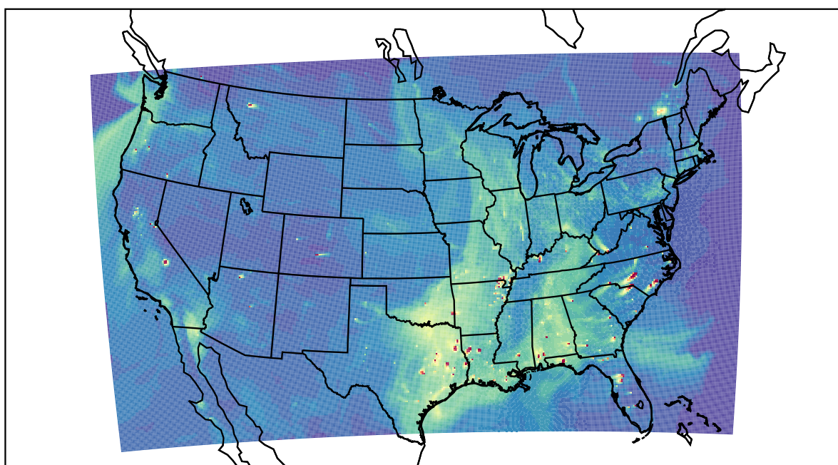
WRF 2019-10-05_22:00:00
