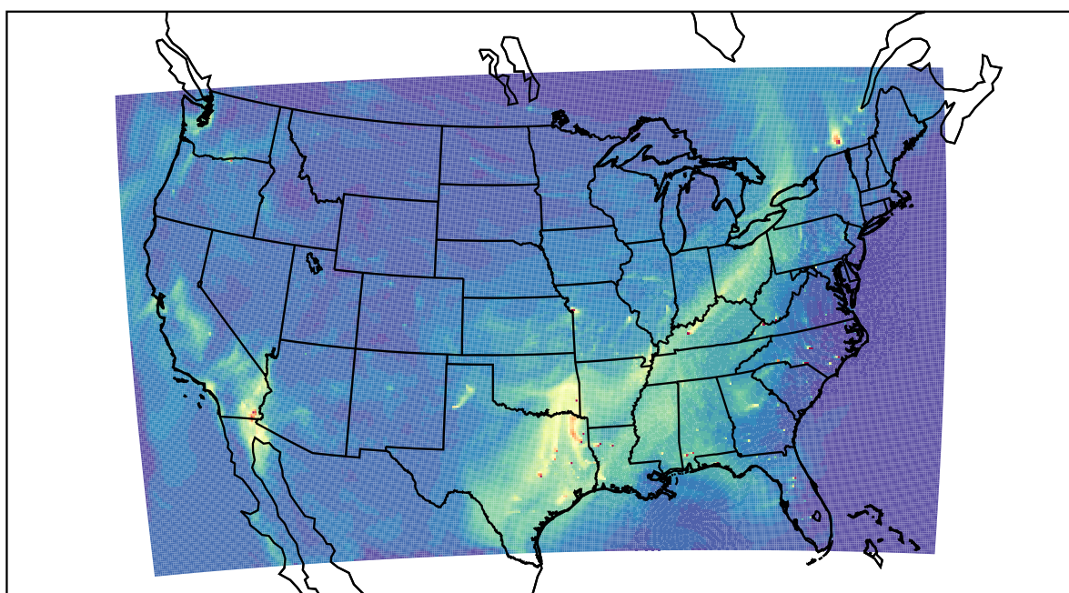
WRF 2019-10-06_18:00:00
