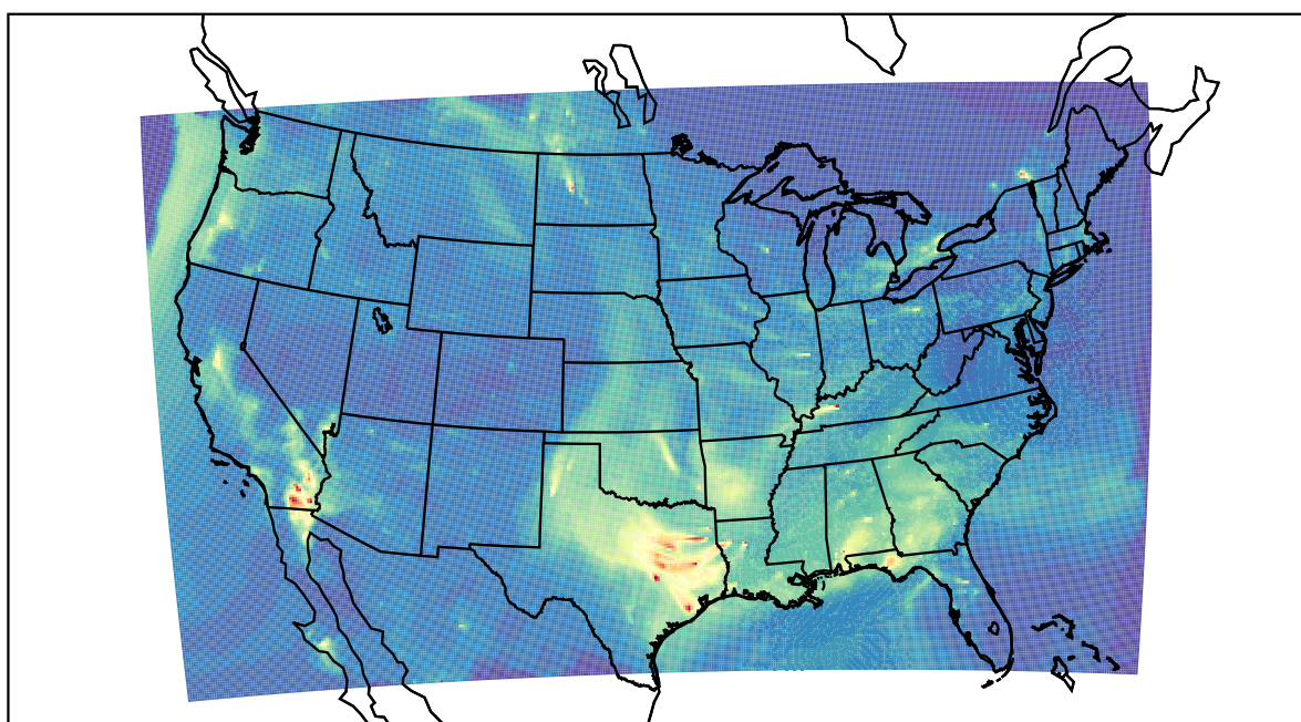
WRF 2019-10-05_10:00:00
