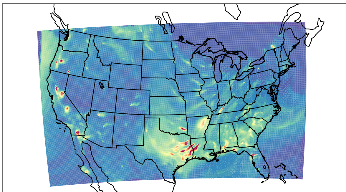
WRF 2019-10-05_04:00:00
