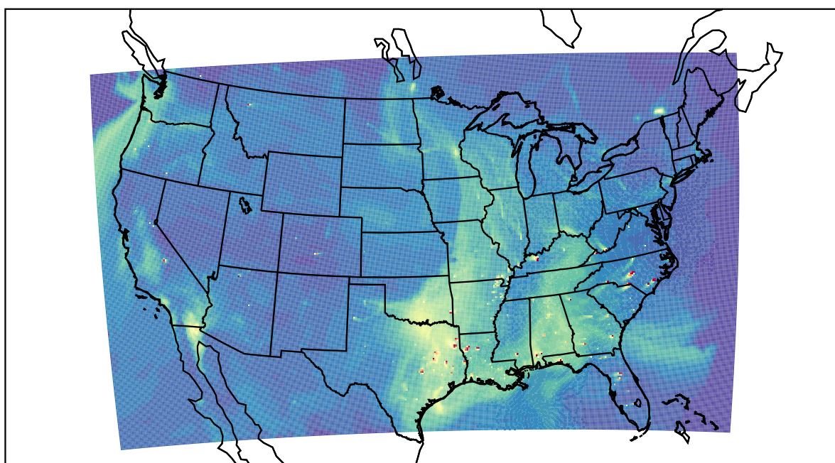
WRF 2019-10-05_20:00:00
