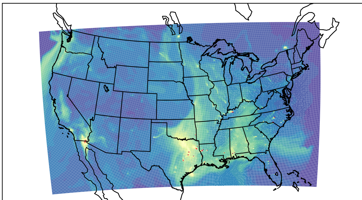
WRF 2019-10-05_18:00:00
