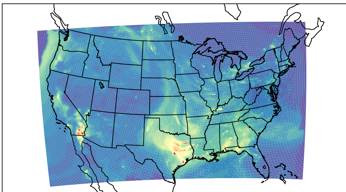
WRF 2019-10-05_11:00:00
