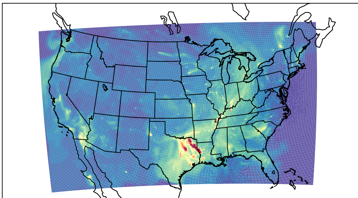
WRF 2019-10-06_10:00:00
