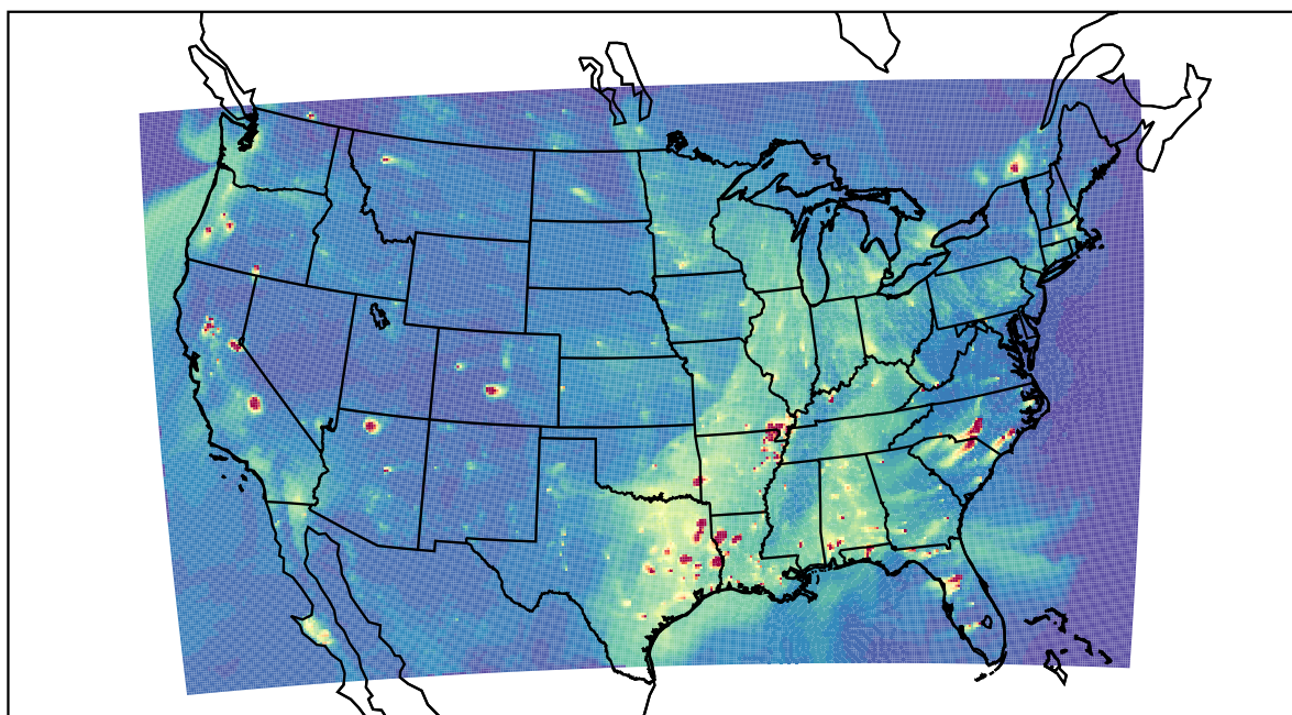
WRF 2019-10-06_01:00:00
