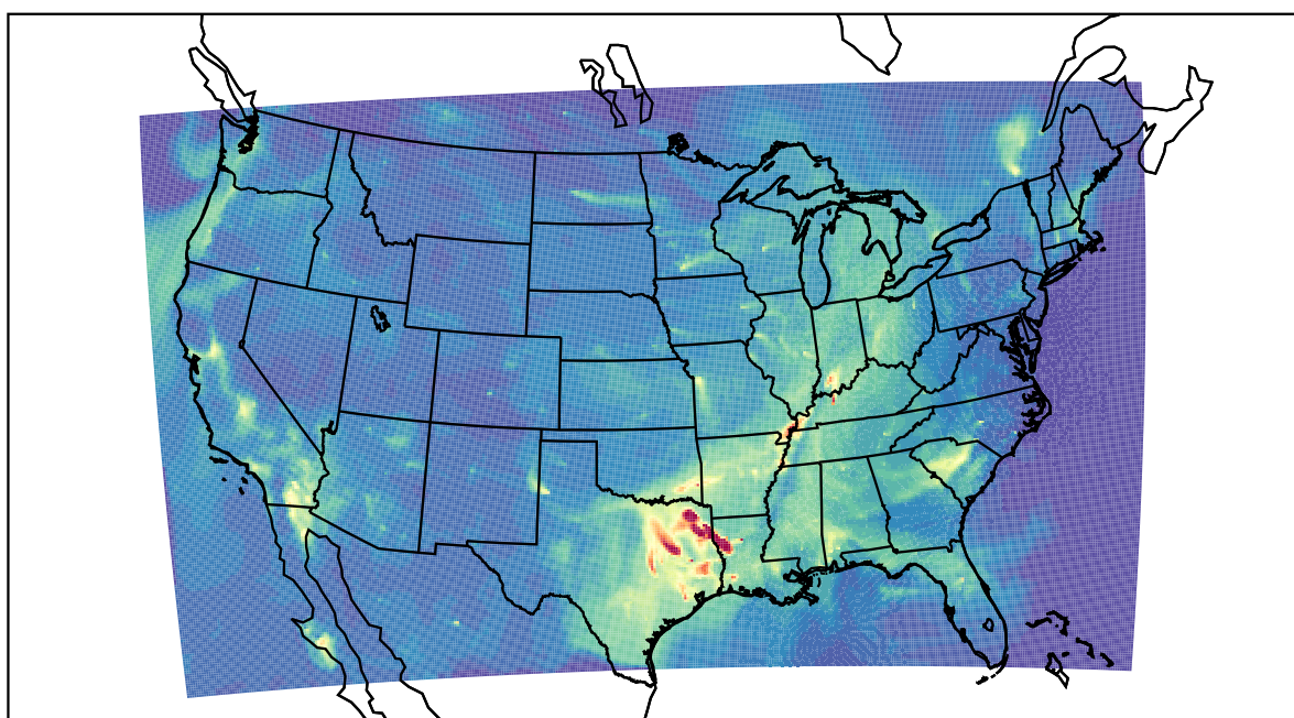
WRF 2019-10-06_08:00:00
