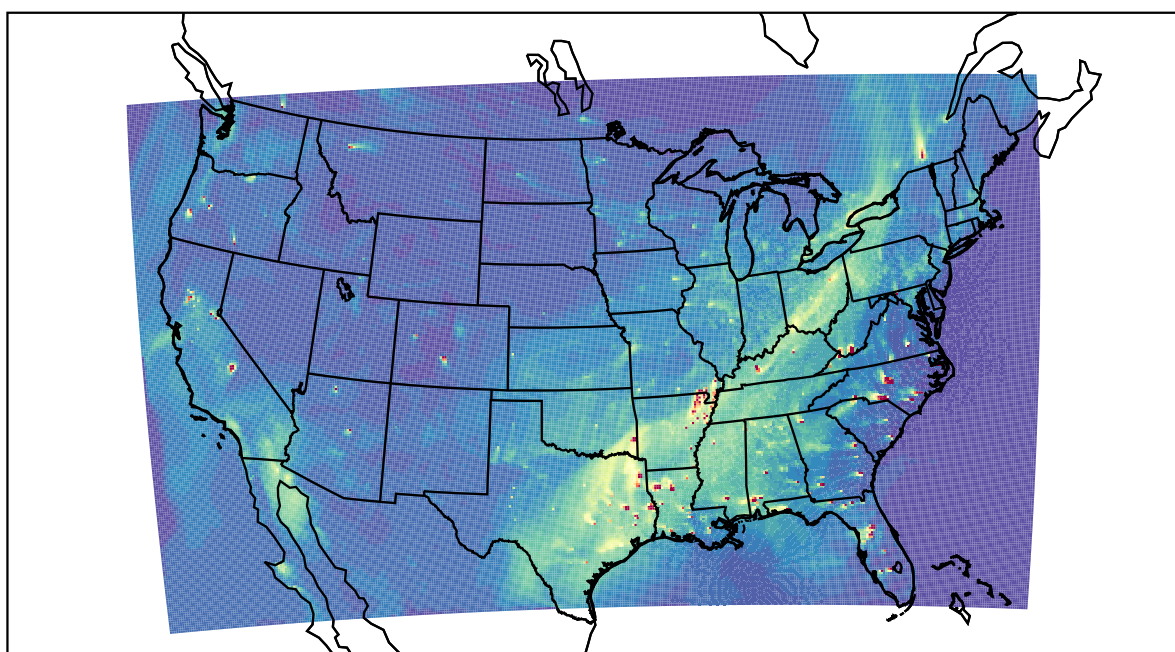
WRF 2019-10-06_23:00:00
