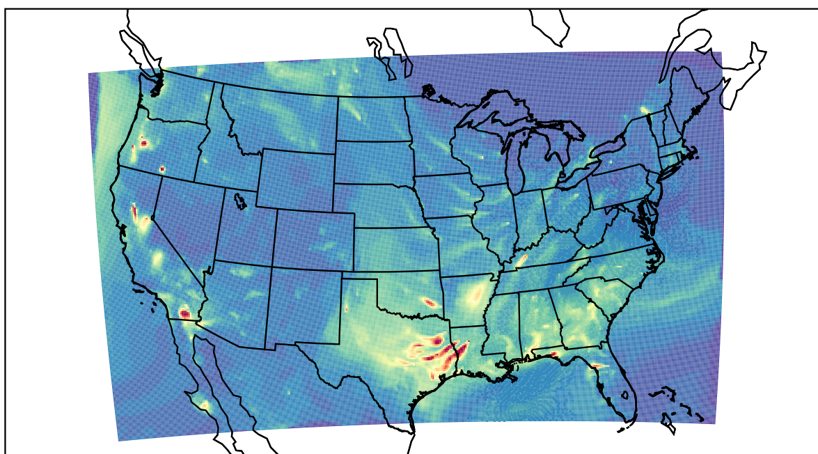
WRF 2019-10-05_05:00:00
