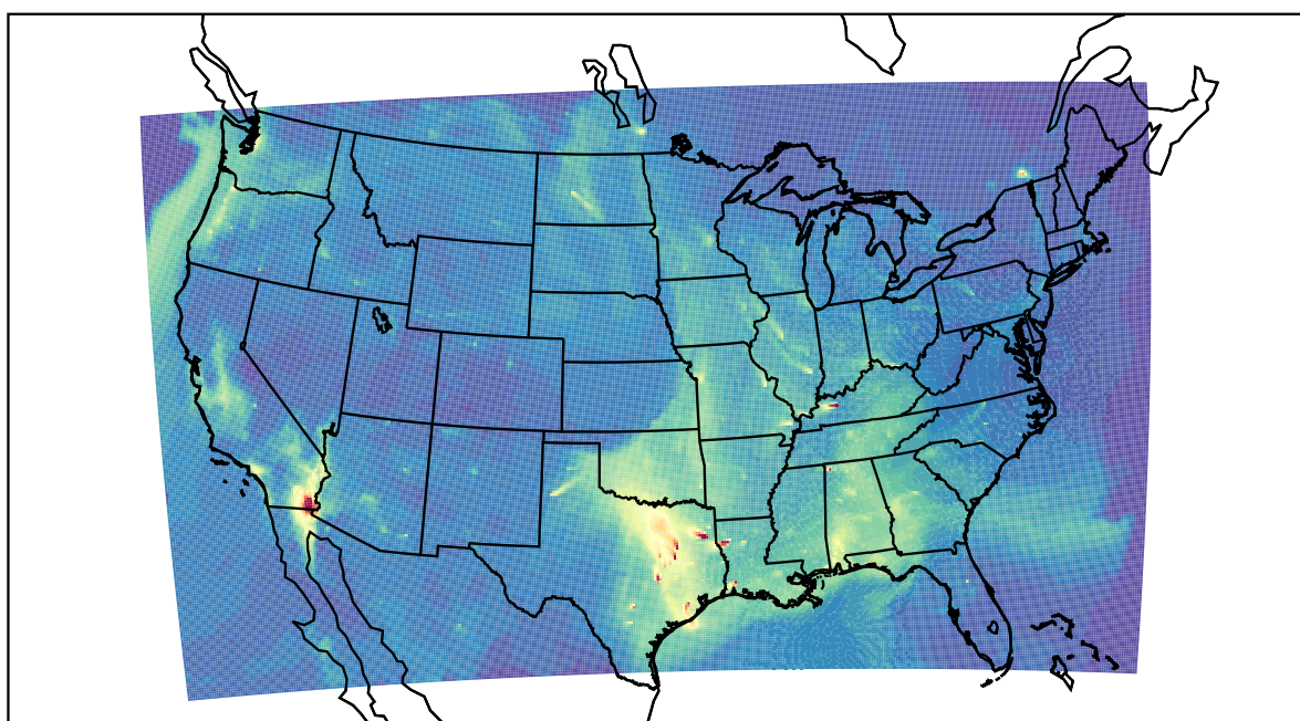
WRF 2019-10-05_16:00:00
