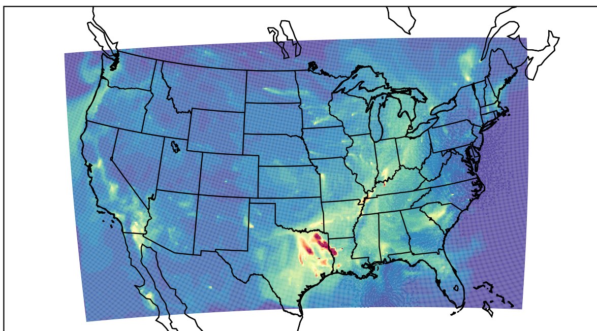
WRF 2019-10-06_09:00:00
