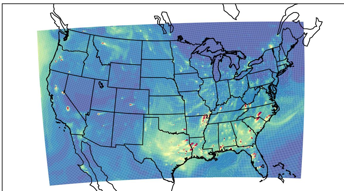
WRF 2019-10-05_00:00:00
