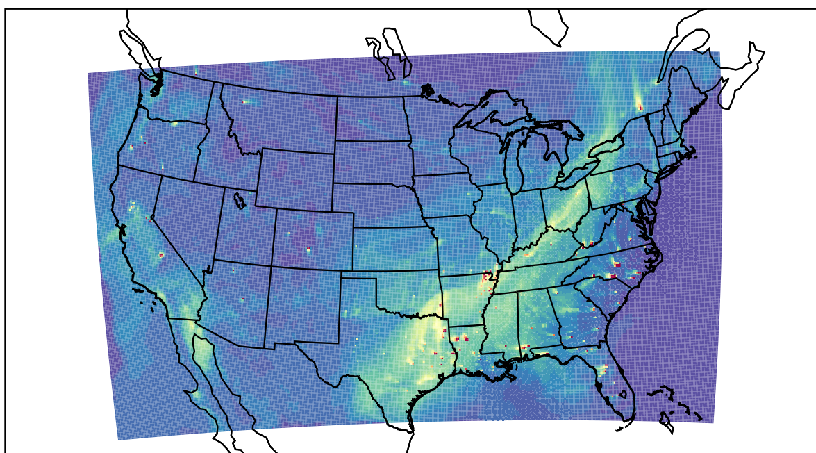
WRF 2019-10-06_22:00:00
