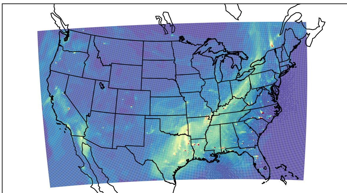
WRF 2019-10-06_21:00:00
