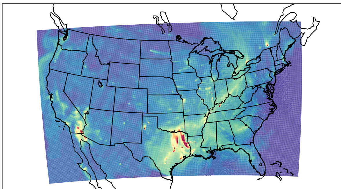
WRF 2019-10-06_14:00:00
