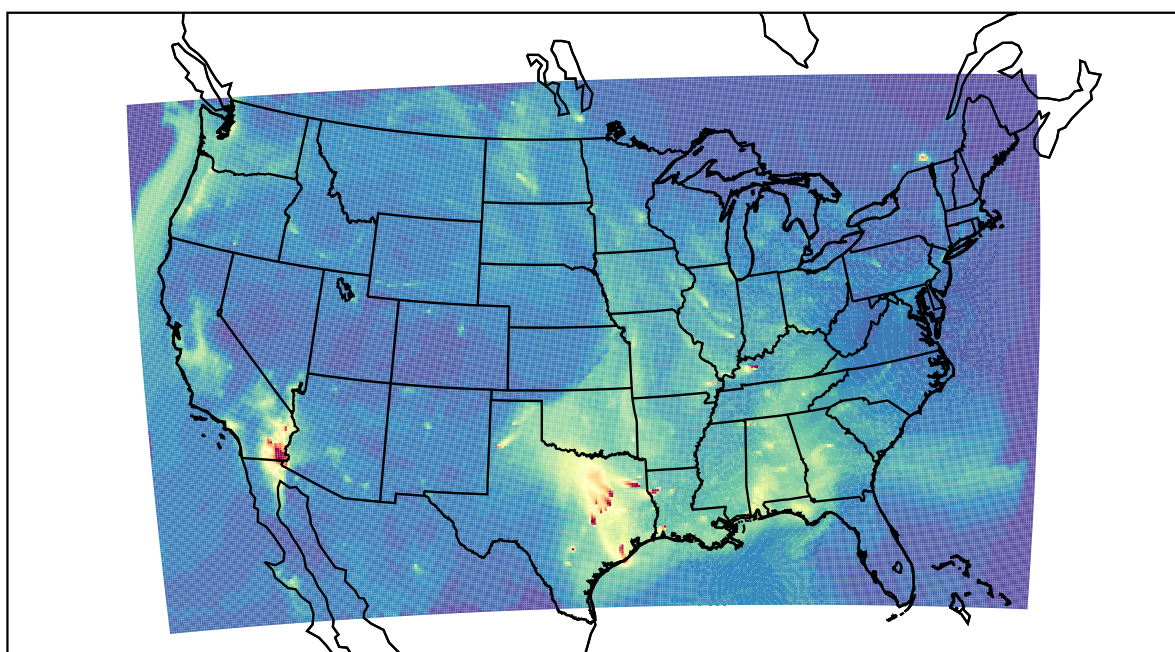
WRF 2019-10-05_15:00:00
