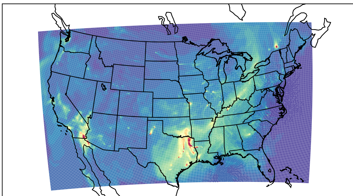
WRF 2019-10-06_16:00:00
