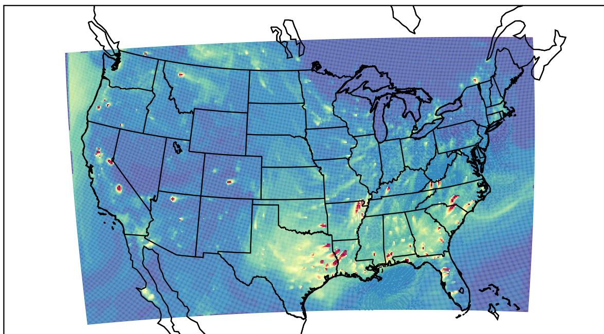
WRF 2019-10-05_01:00:00
