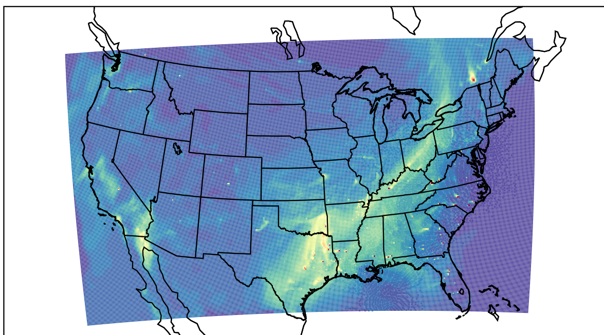
WRF 2019-10-06_19:00:00
