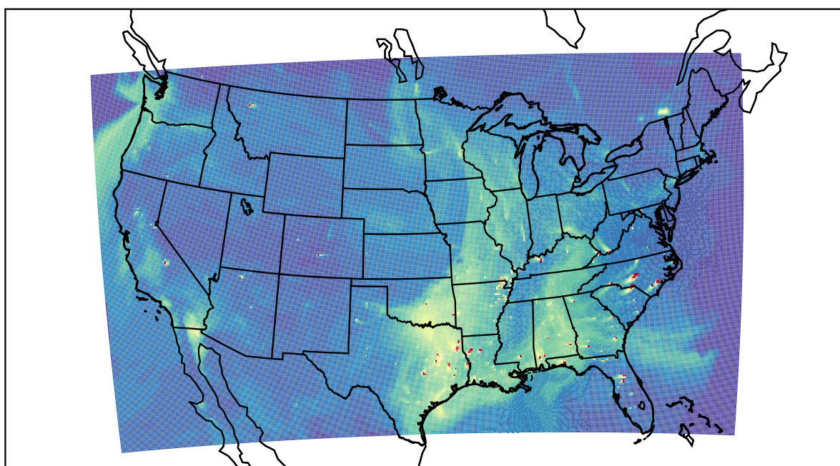
WRF 2019-10-05_21:00:00
