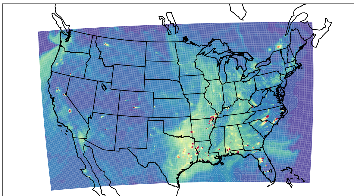
WRF 2019-10-05_23:00:00
