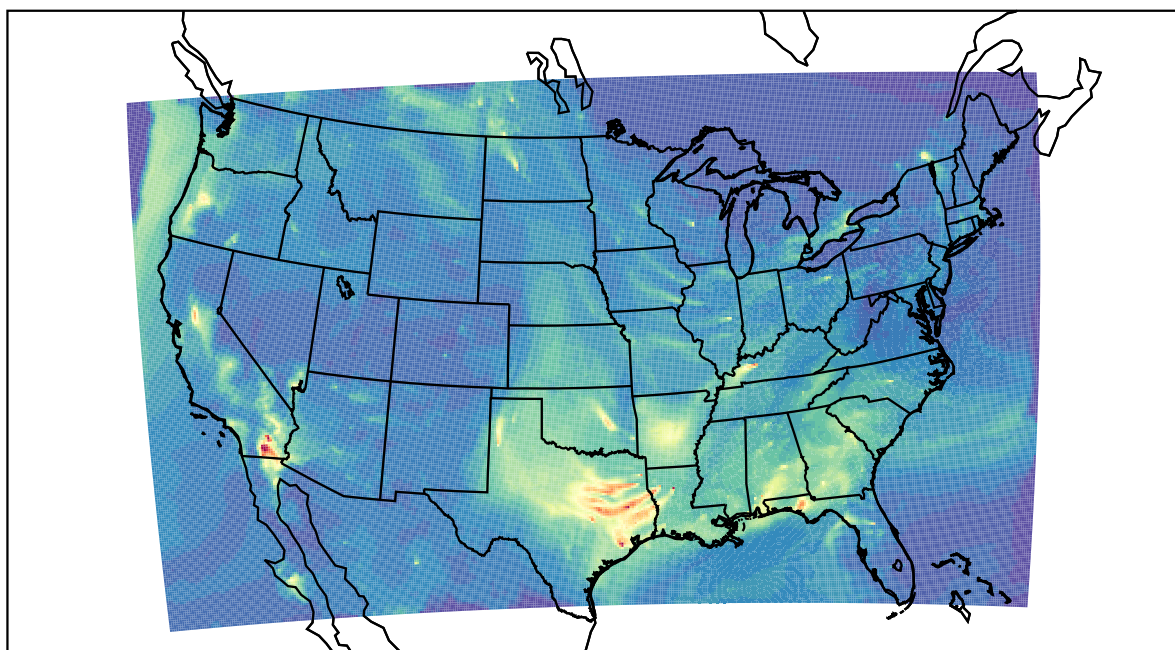
WRF 2019-10-05_08:00:00
