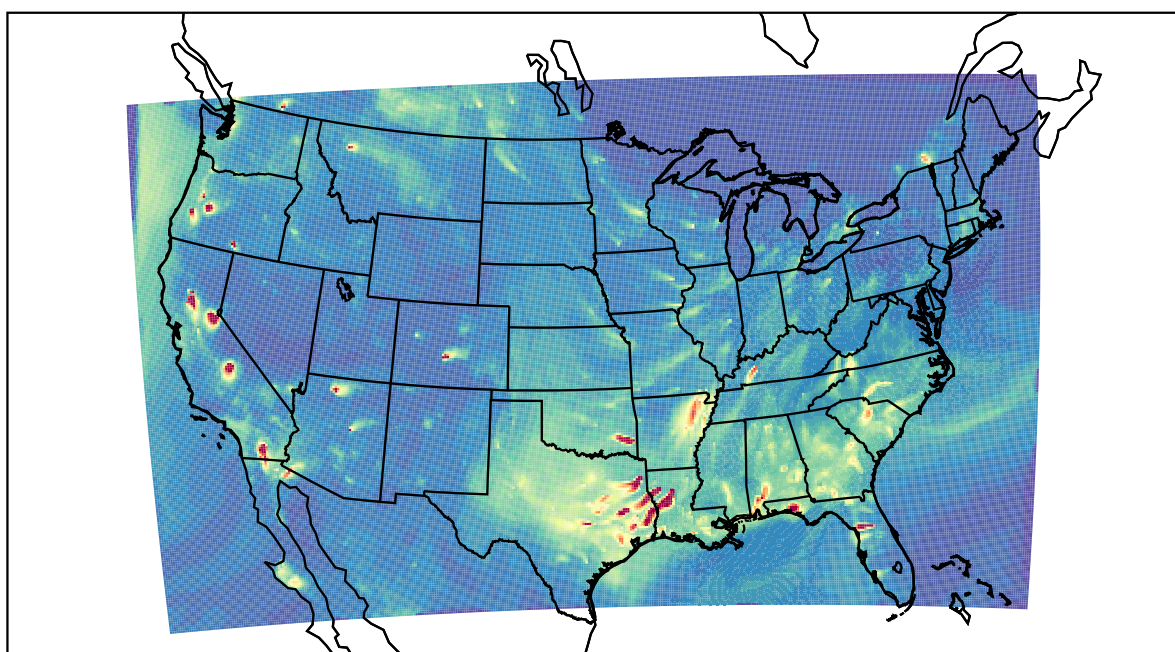
WRF 2019-10-05_03:00:00
