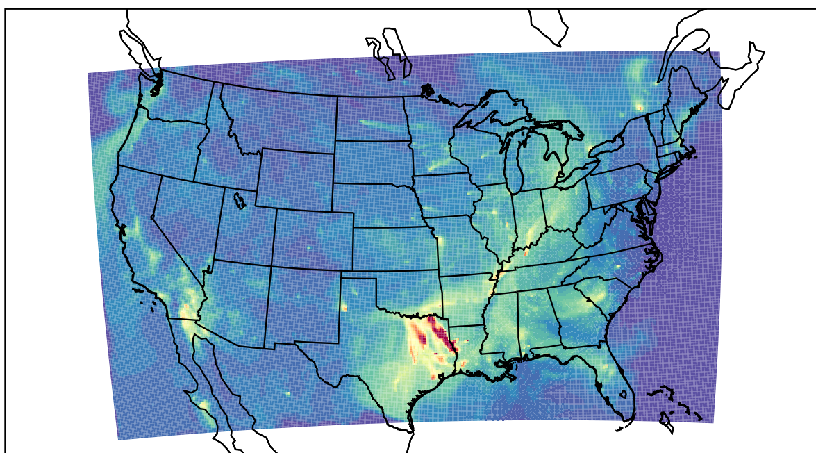
WRF 2019-10-06_11:00:00
