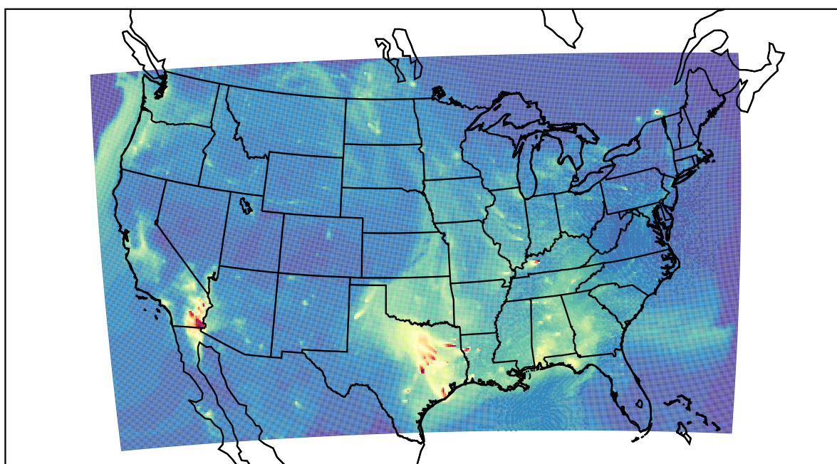
WRF 2019-10-05_14:00:00
