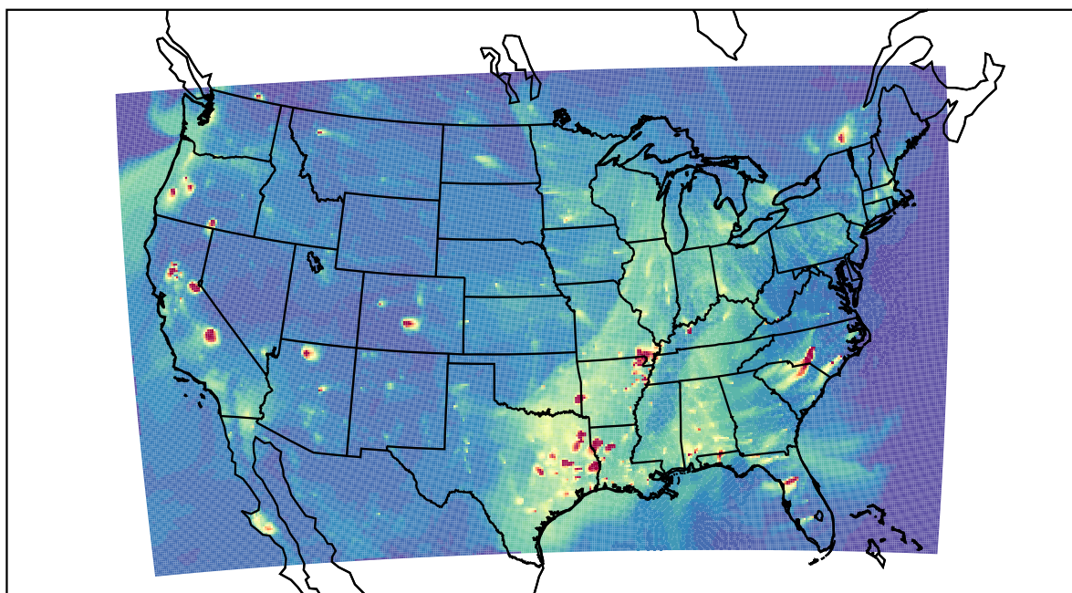
WRF 2019-10-06_02:00:00
