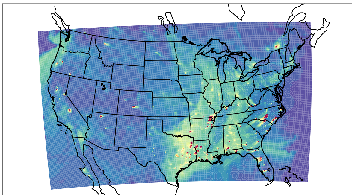
WRF 2019-10-06_00:00:00
