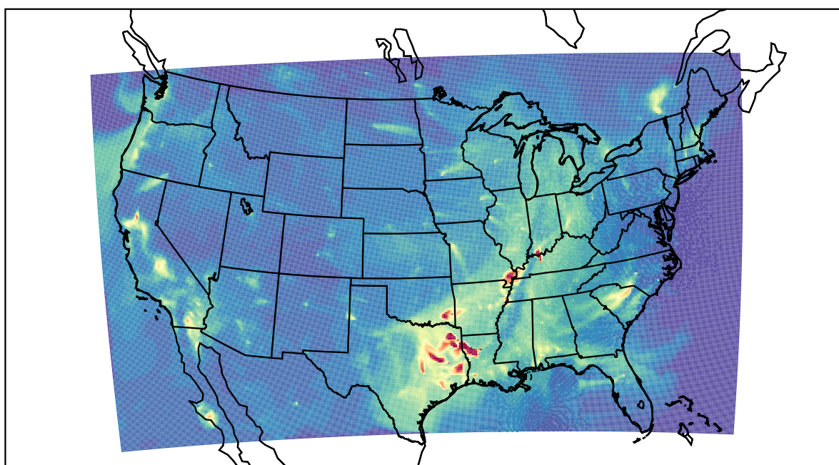
WRF 2019-10-06_06:00:00
