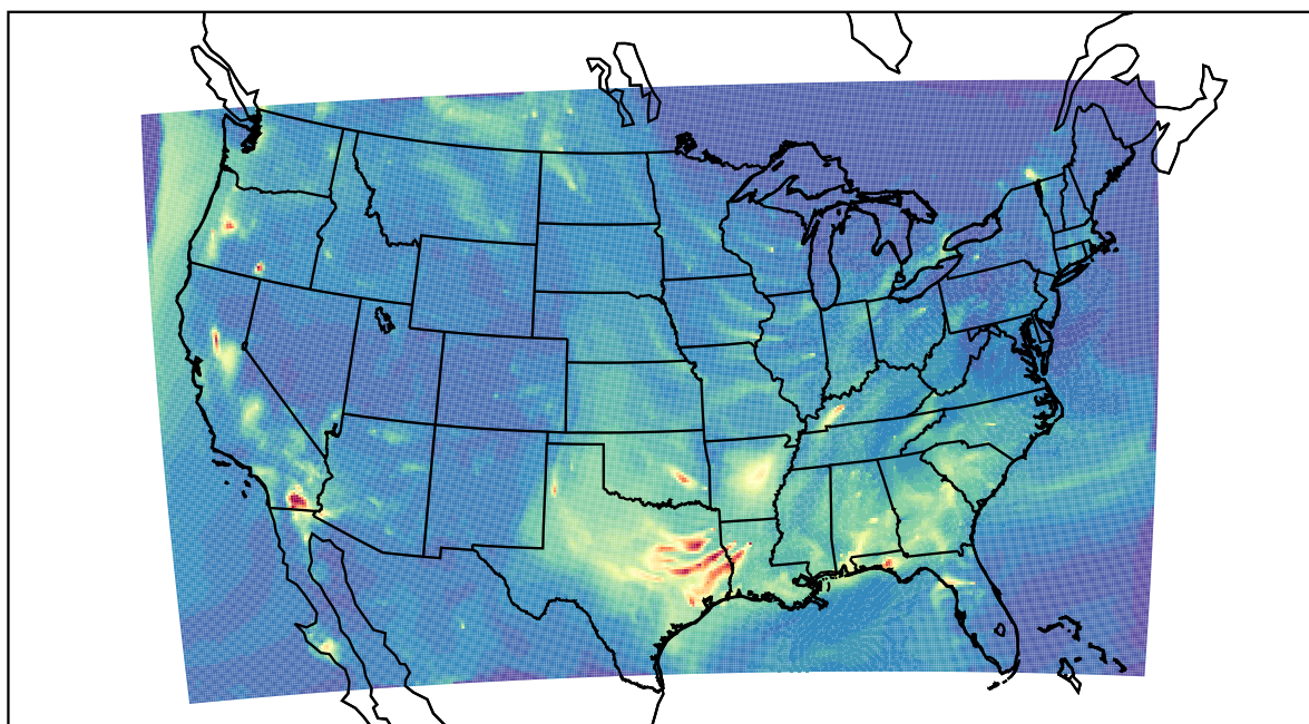
WRF 2019-10-05_06:00:00
