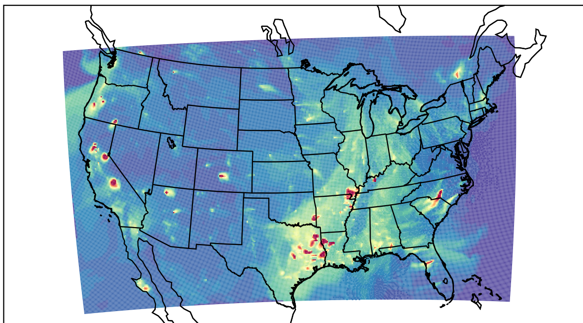
WRF 2019-10-06_03:00:00
