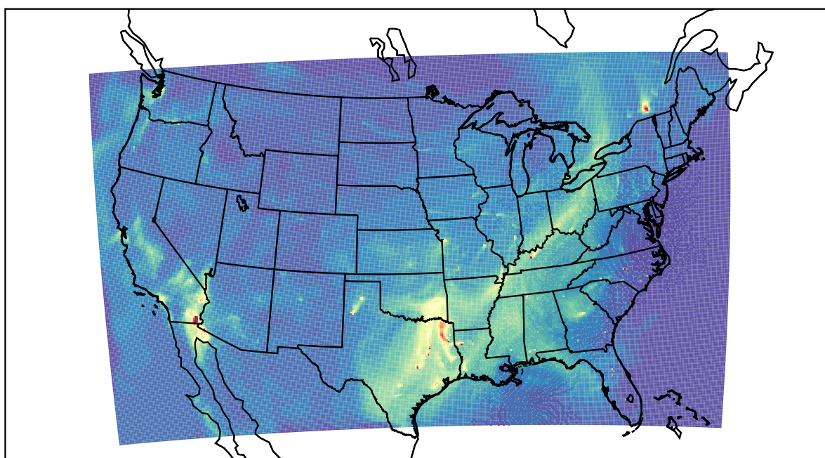
WRF 2019-10-06_17:00:00
