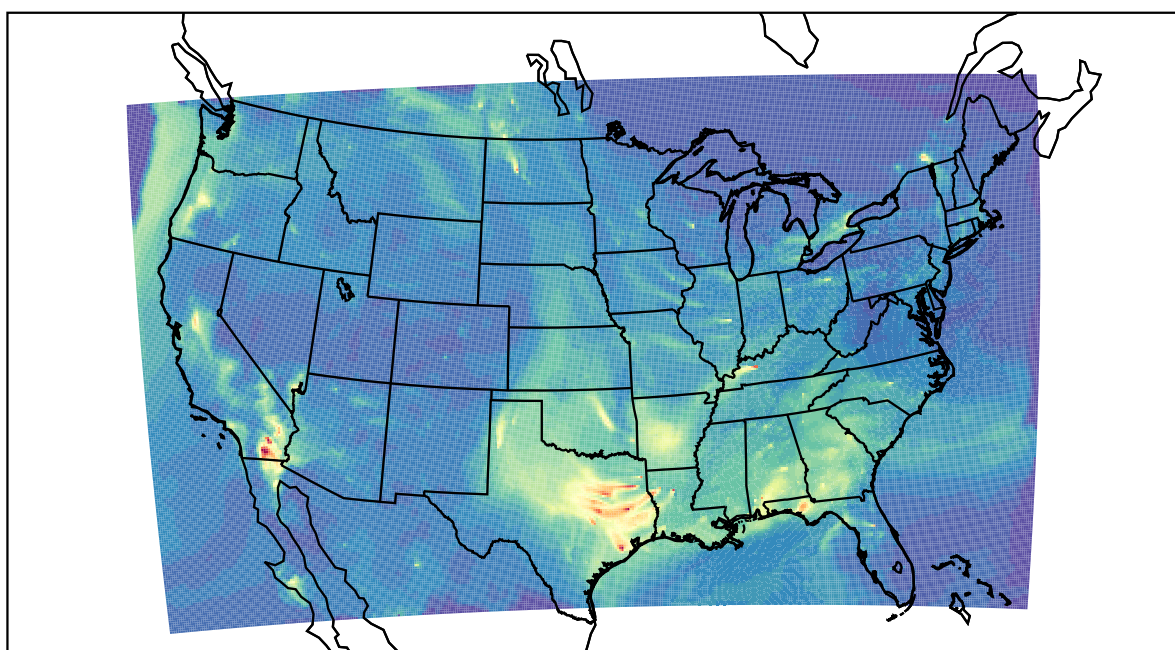
WRF 2019-10-05_09:00:00
