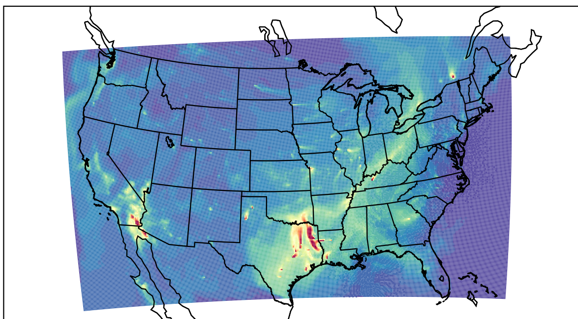
WRF 2019-10-06_15:00:00
