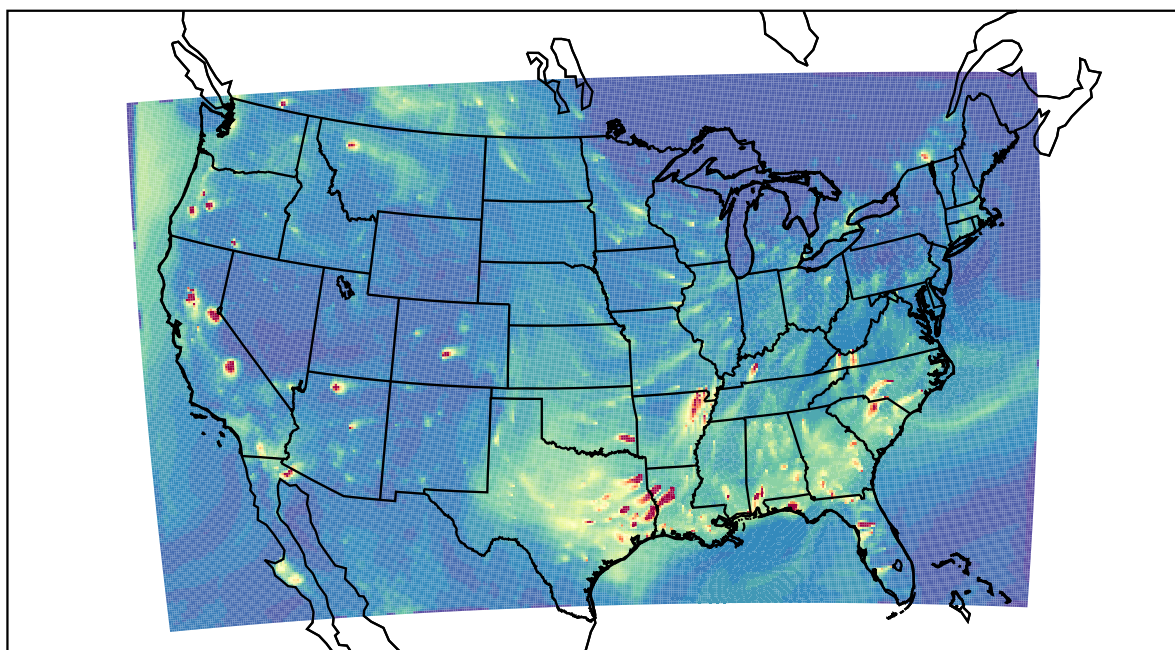
WRF 2019-10-05_02:00:00
