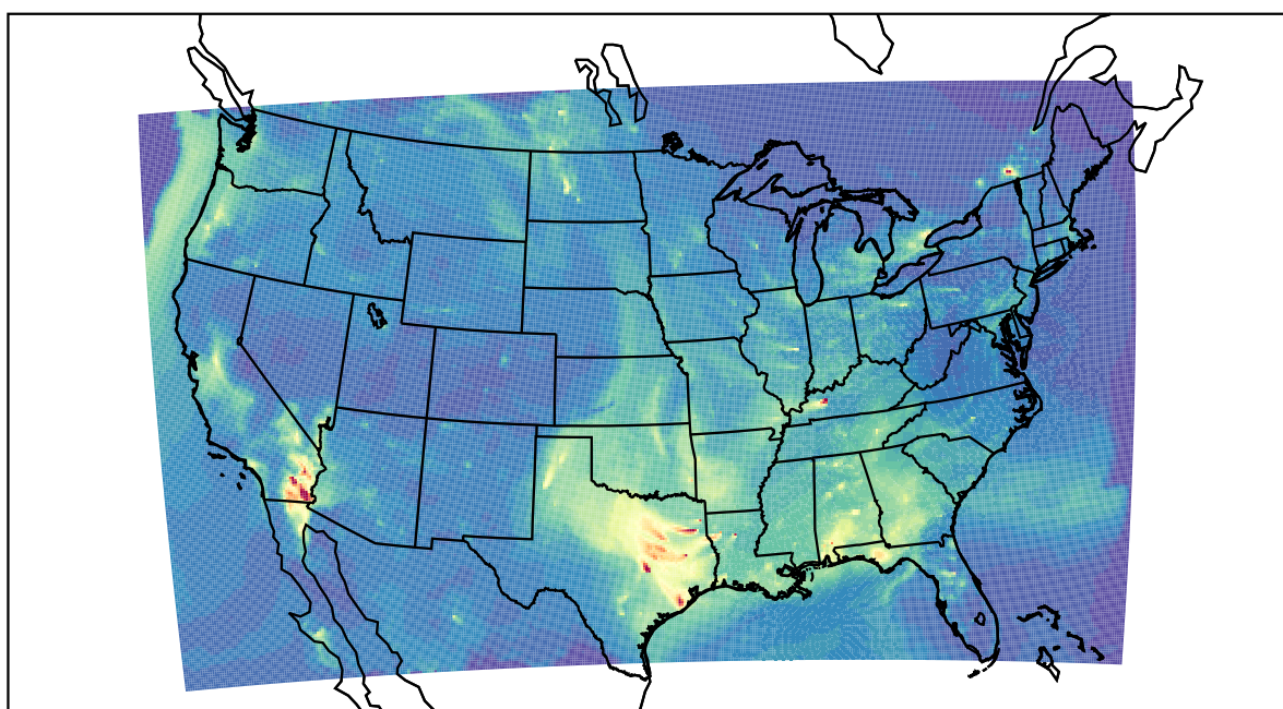
WRF 2019-10-05_12:00:00
