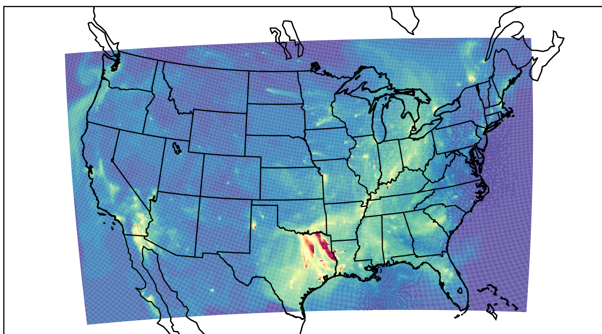
WRF 2019-10-06_12:00:00
