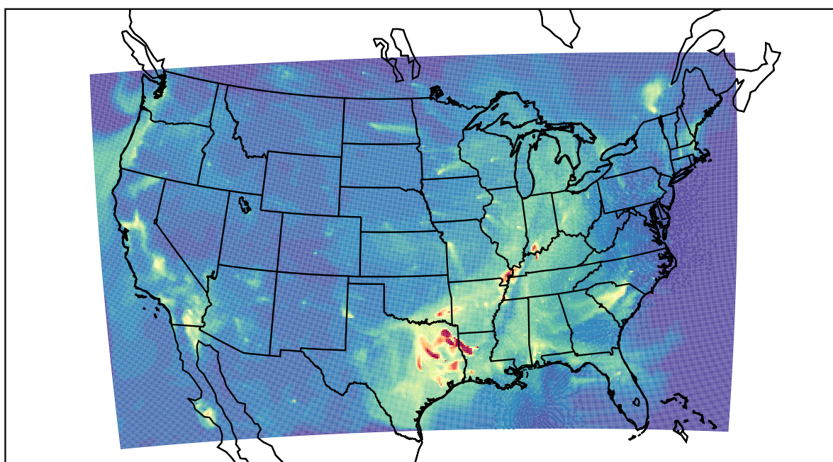
WRF 2019-10-06_07:00:00
