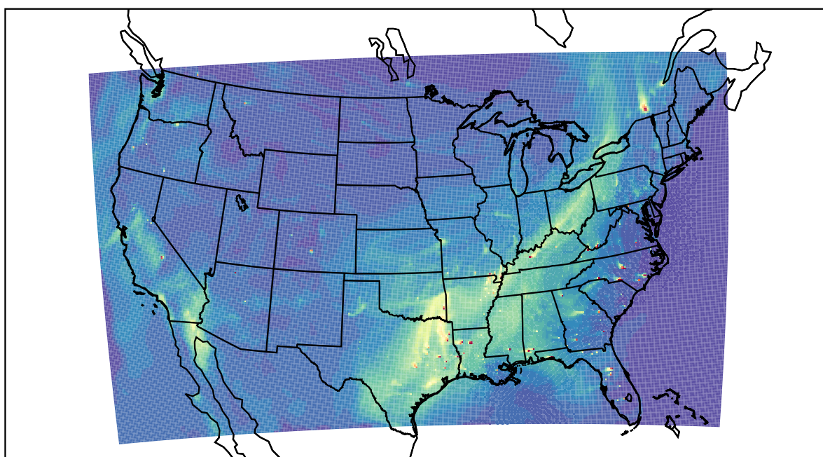
WRF 2019-10-06_20:00:00
