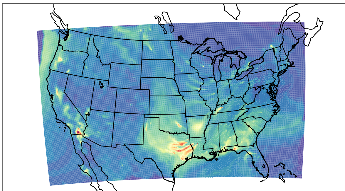
WRF 2019-10-05_07:00:00
