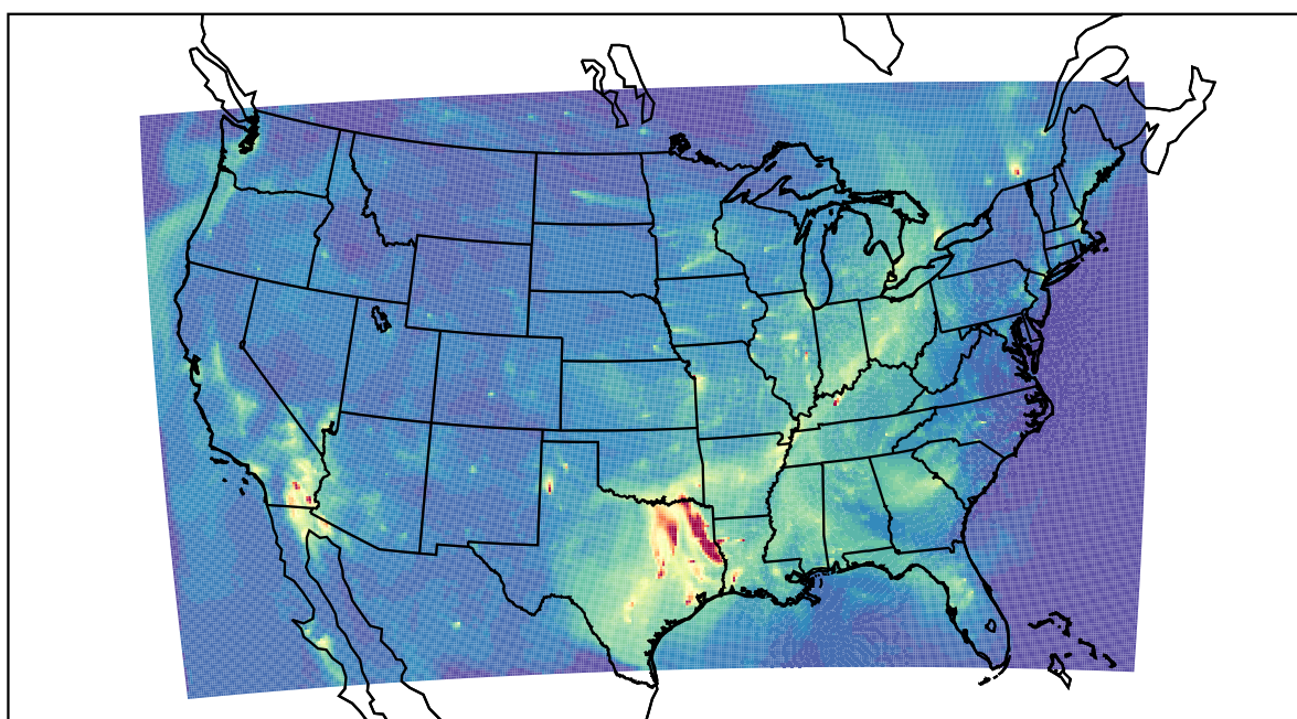
WRF 2019-10-06_13:00:00
