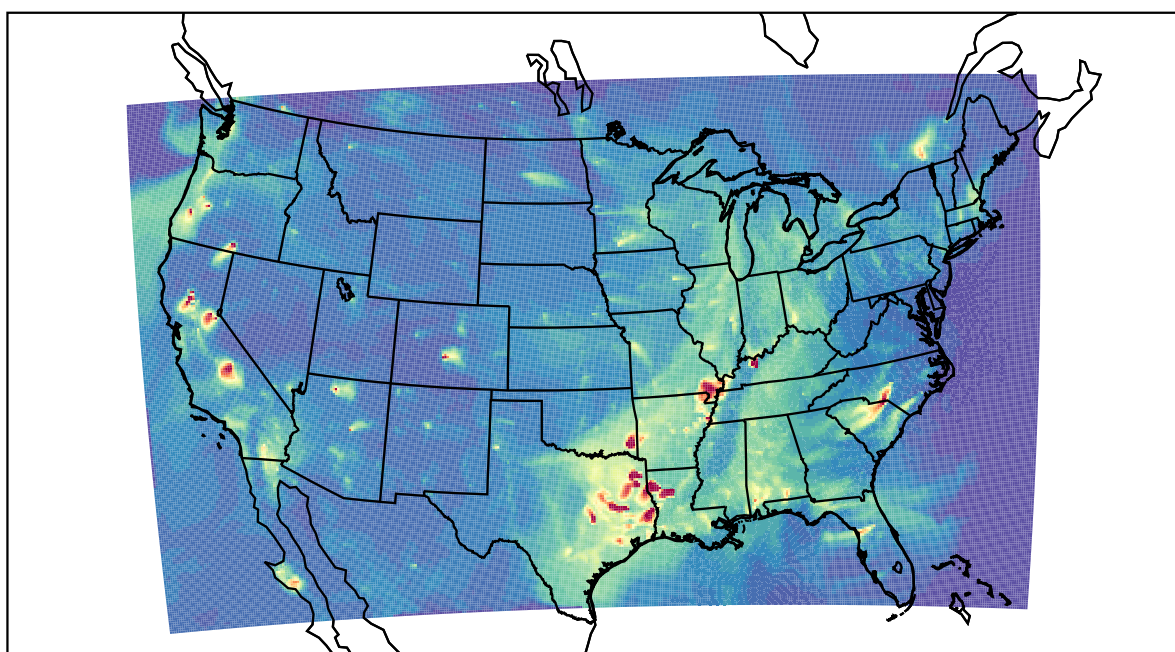
WRF 2019-10-06_04:00:00
