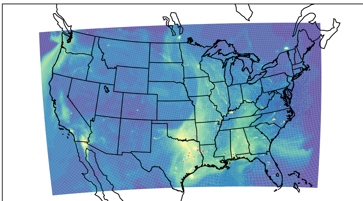
WRF 2019-10-05_19:00:00
