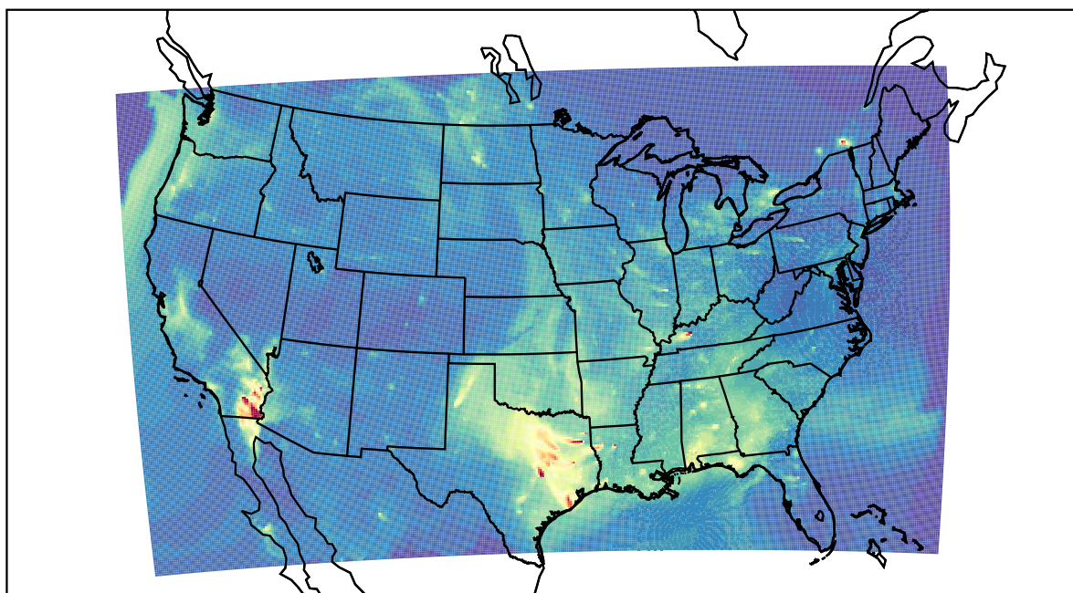
WRF 2019-10-05_13:00:00
