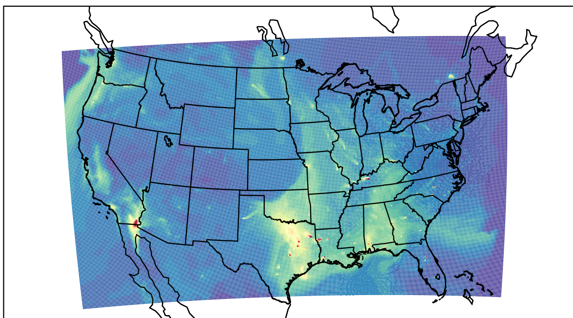
WRF 2019-10-05_17:00:00
