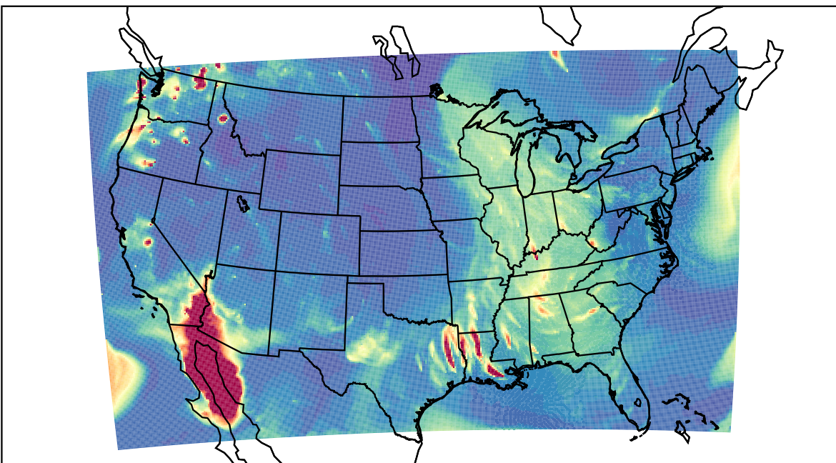
WRF 2019-10-11_04:00:00
