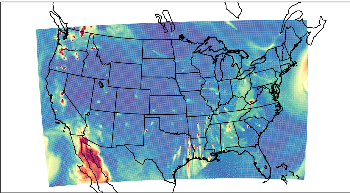
WRF 2019-10-12_03:00:00
