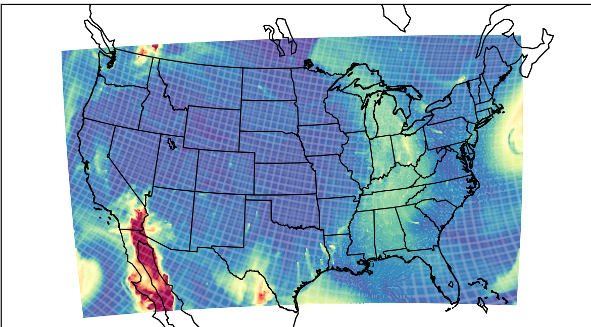
WRF 2019-10-11_16:00:00
