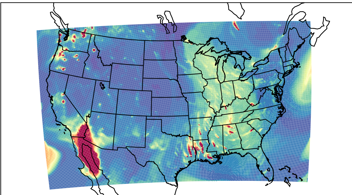
WRF 2019-10-11_02:00:00
