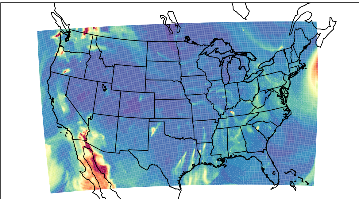
WRF 2019-10-12_08:00:00
