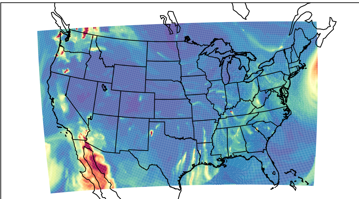
WRF 2019-10-12_06:00:00
