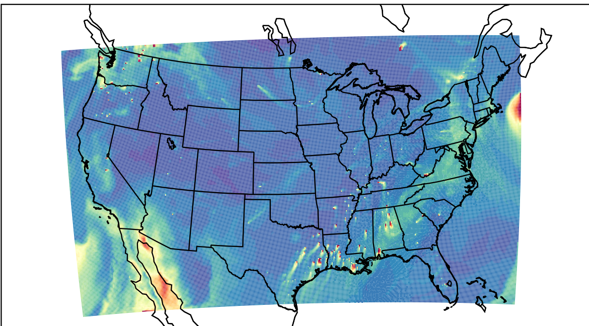
WRF 2019-10-12_21:00:00
