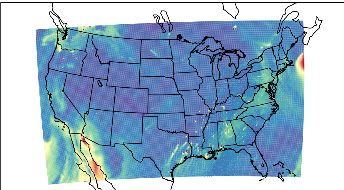
WRF 2019-10-12_20:00:00
