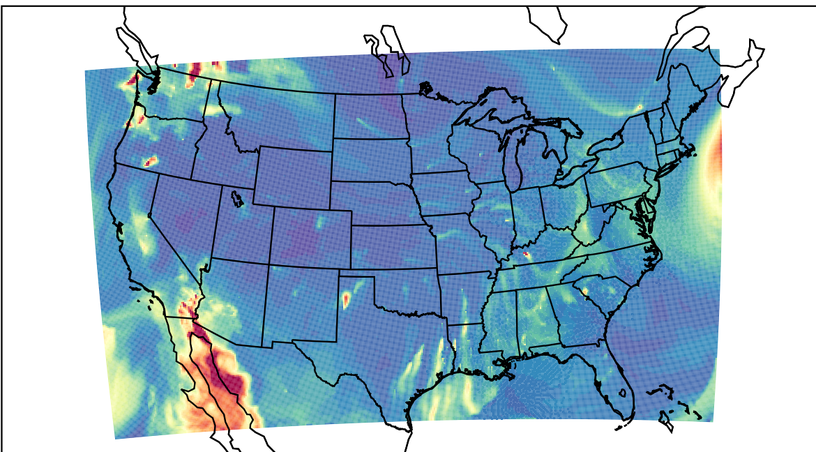
WRF 2019-10-12_07:00:00
