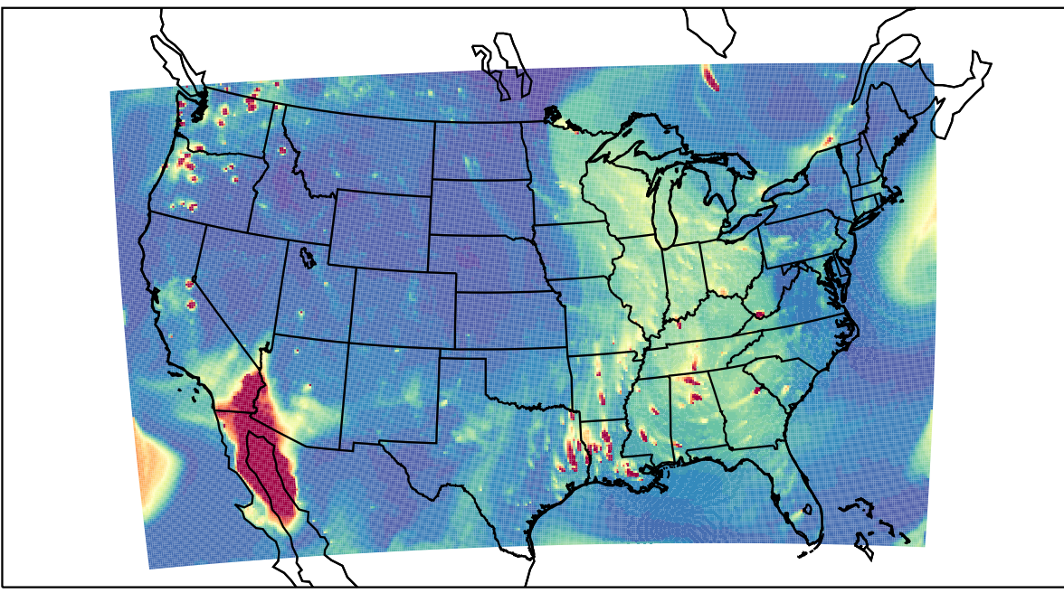
WRF 2019-10-11_01:00:00
