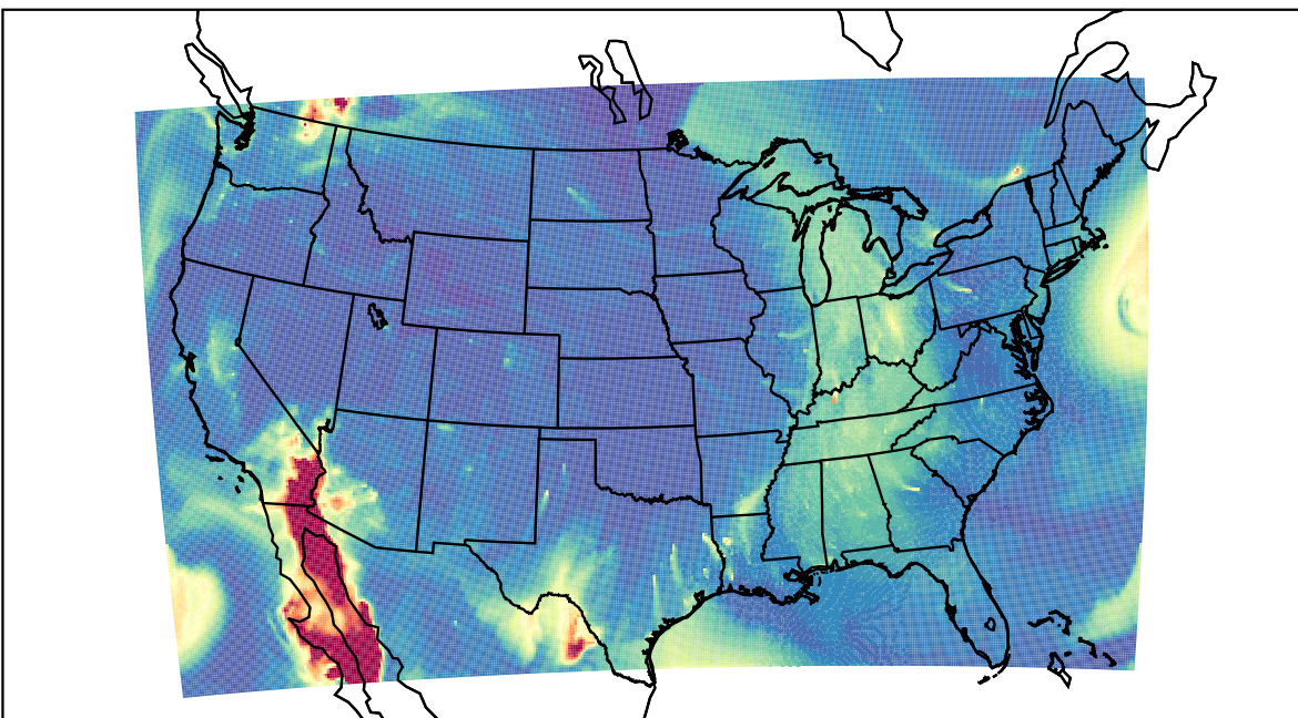
WRF 2019-10-11_15:00:00
