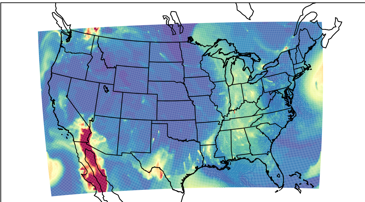
WRF 2019-10-11_13:00:00
