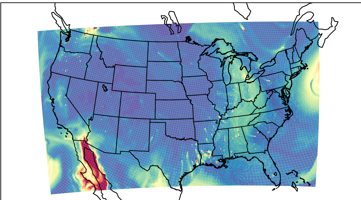
WRF 2019-10-11_20:00:00
