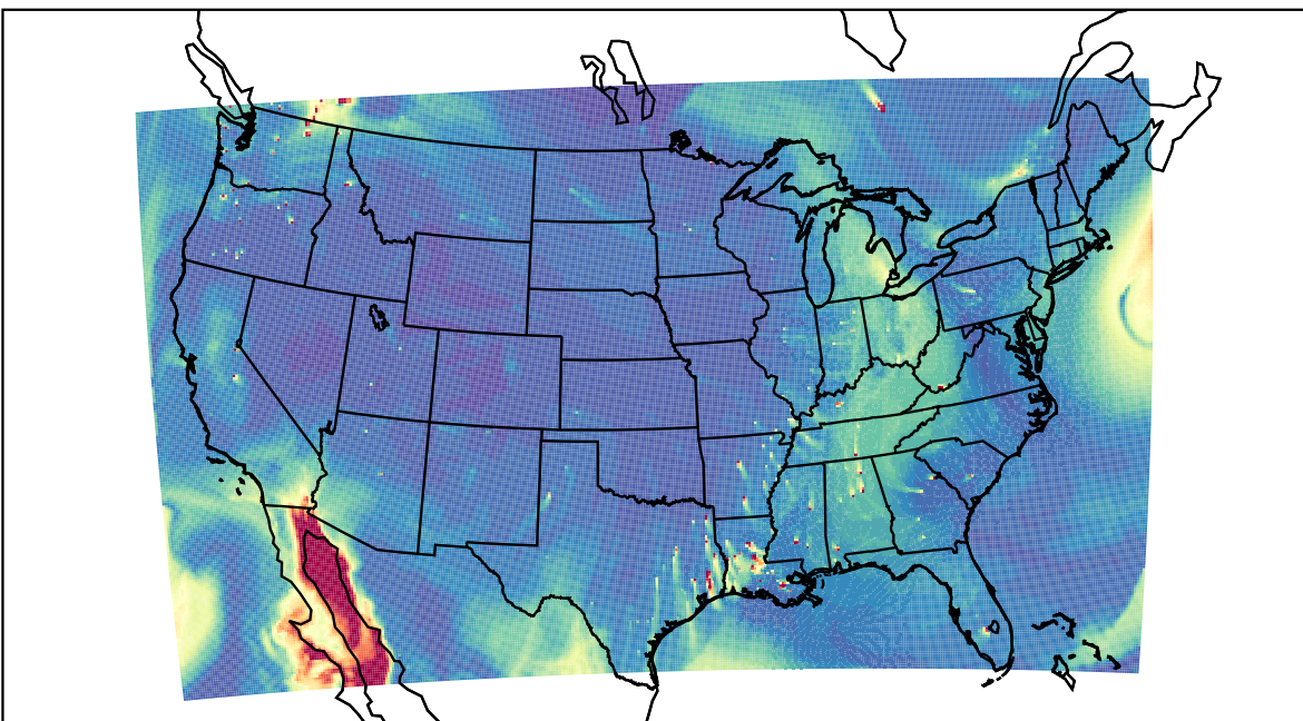
WRF 2019-10-11_21:00:00
