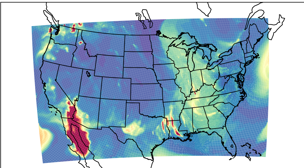
WRF 2019-10-11_06:00:00
