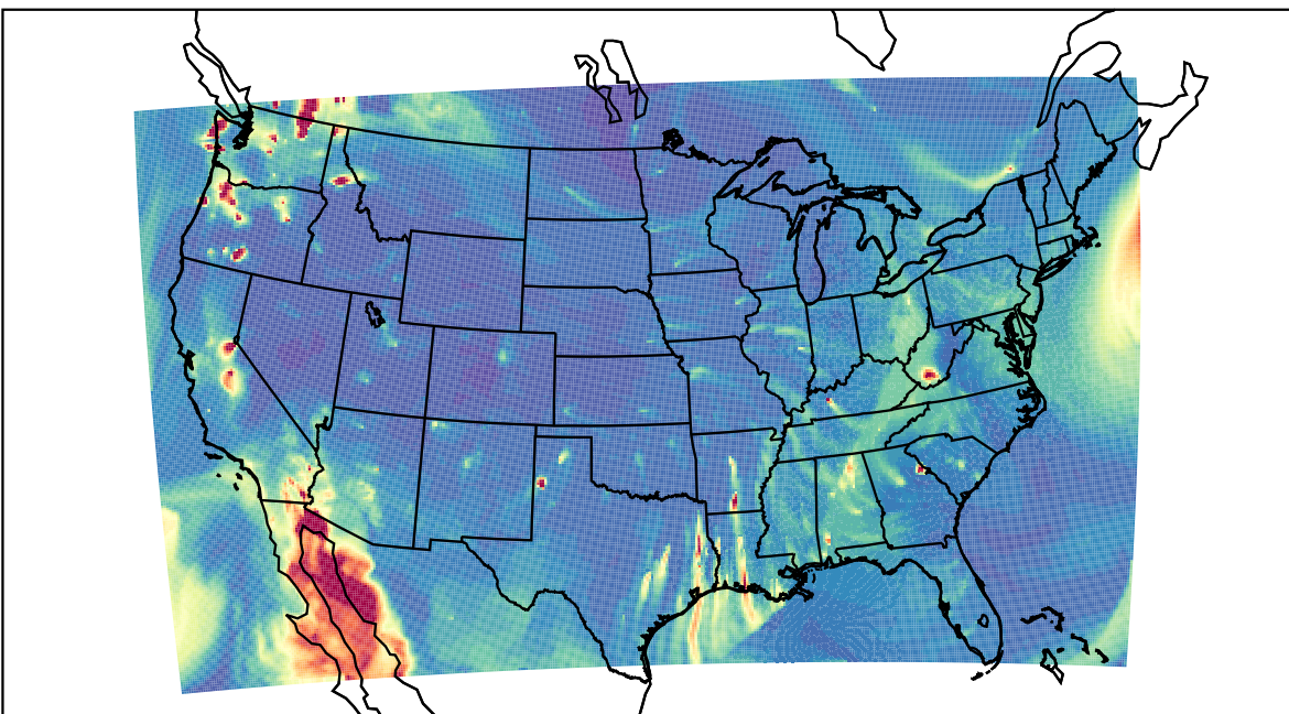
WRF 2019-10-12_04:00:00
