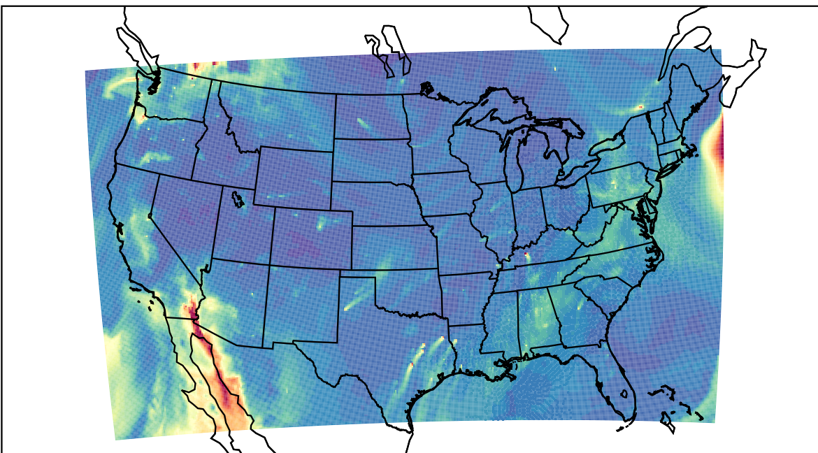
WRF 2019-10-12_16:00:00
