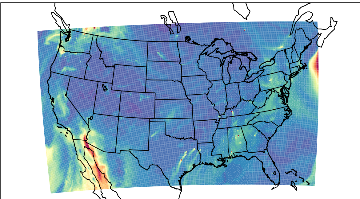
WRF 2019-10-12_17:00:00
