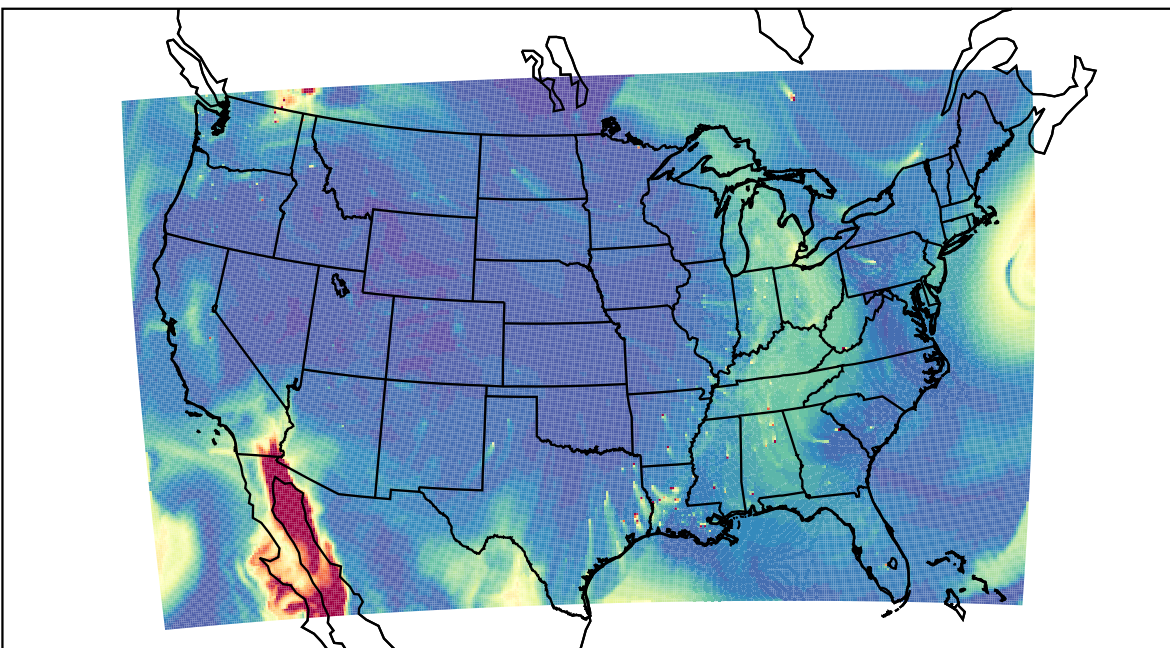
WRF 2019-10-11_19:00:00
