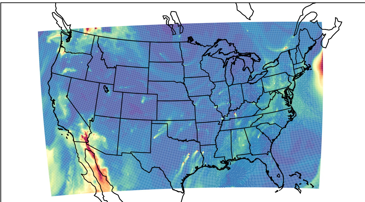
WRF 2019-10-12_15:00:00
