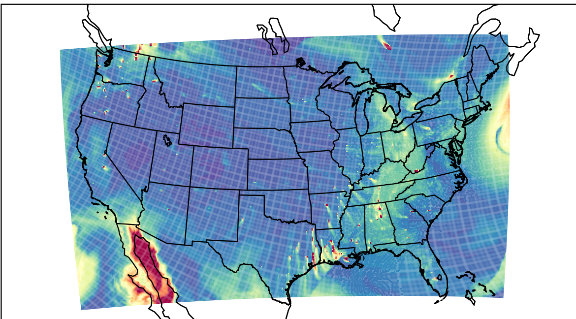
WRF 2019-10-11_23:00:00
