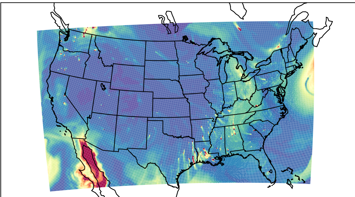
WRF 2019-10-11_22:00:00
