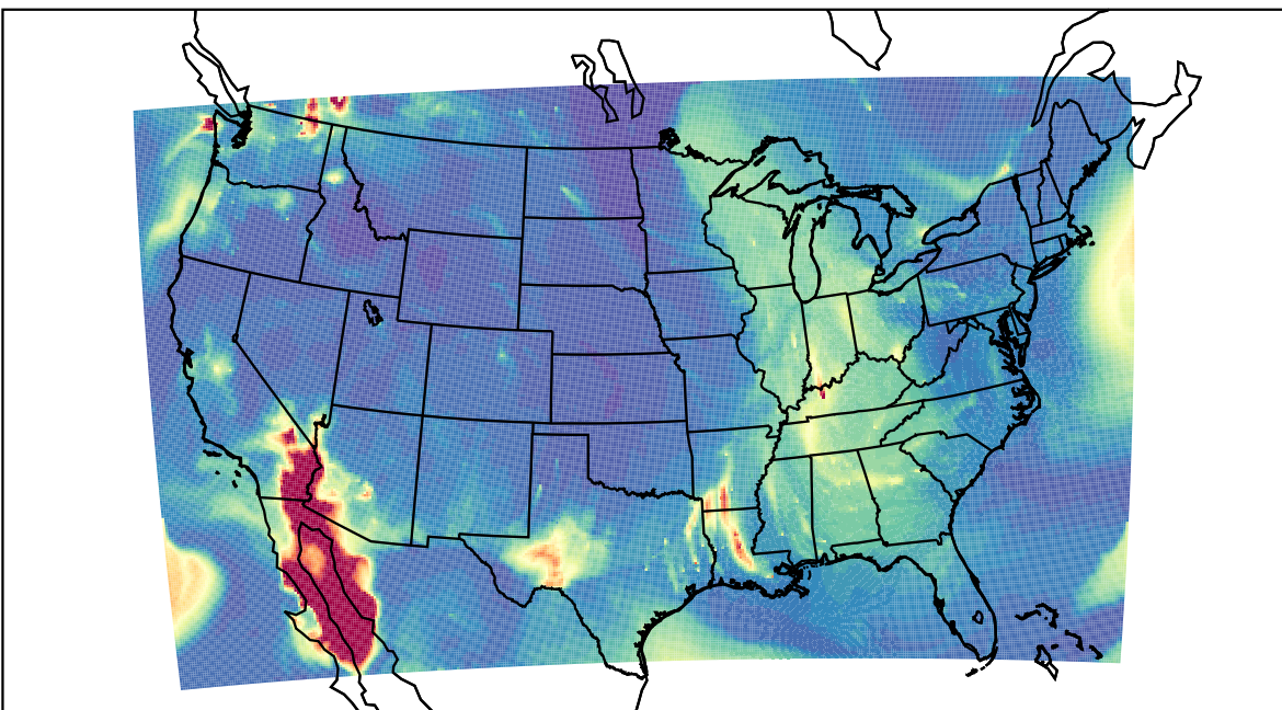
WRF 2019-10-11_08:00:00
