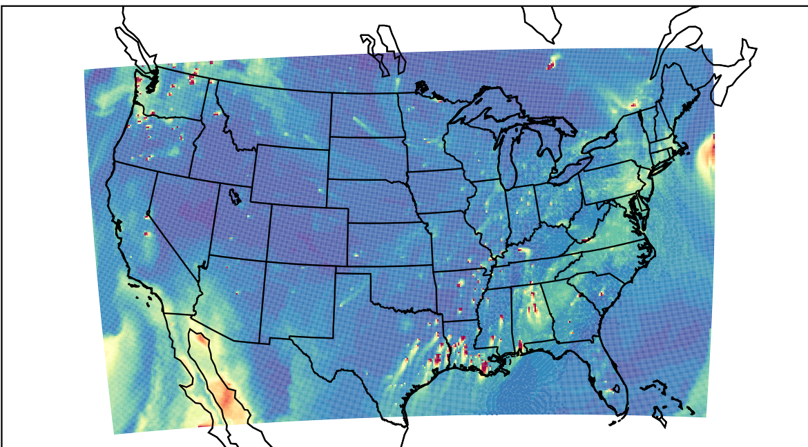
WRF 2019-10-12_23:00:00
