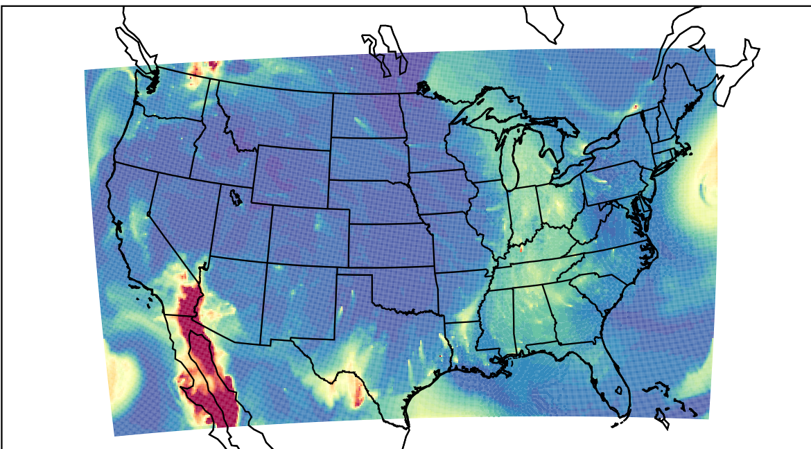
WRF 2019-10-11_14:00:00
