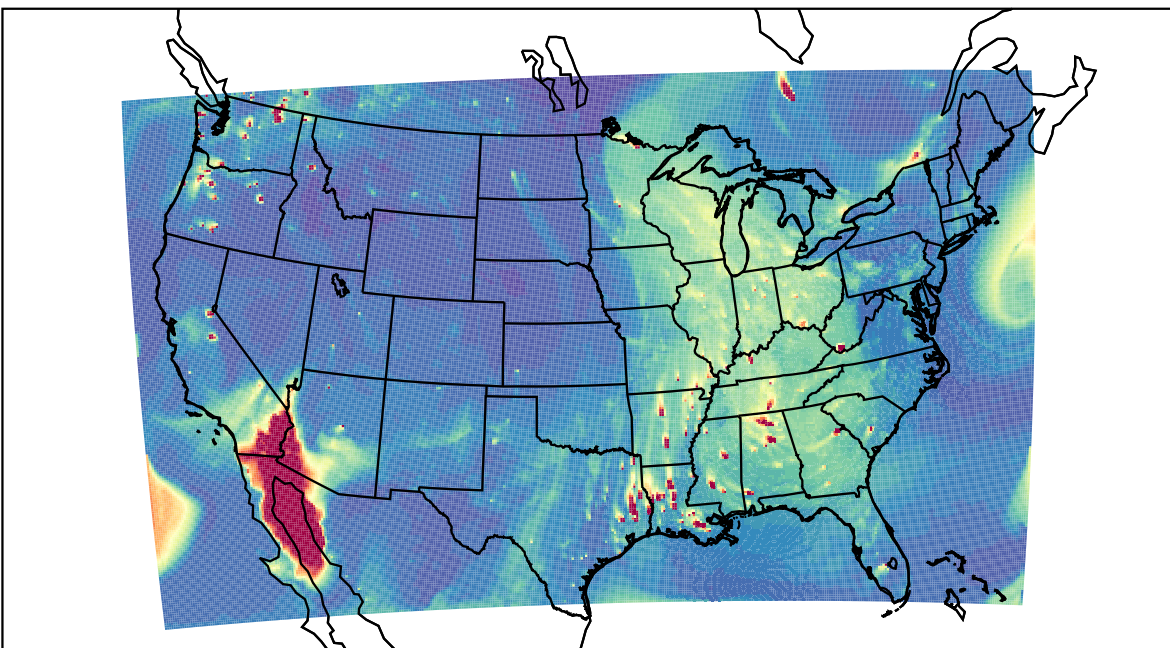
WRF 2019-10-11_00:00:00
