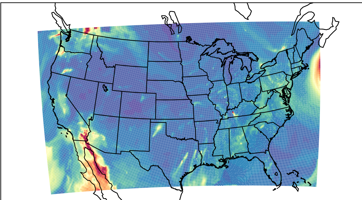
WRF 2019-10-12_11:00:00
