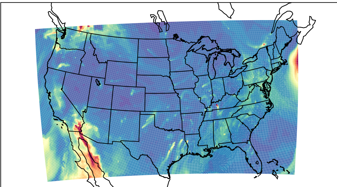
WRF 2019-10-12_14:00:00
