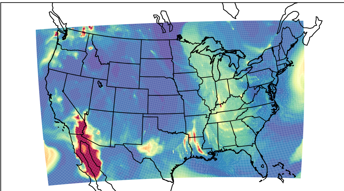
WRF 2019-10-11_07:00:00
