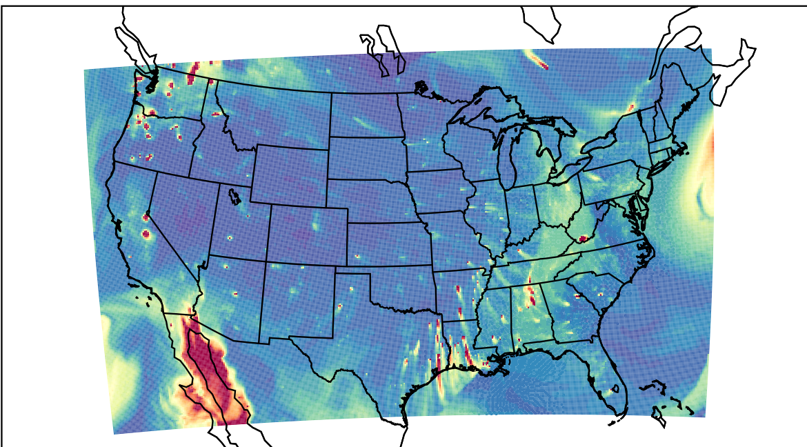
WRF 2019-10-12_01:00:00
