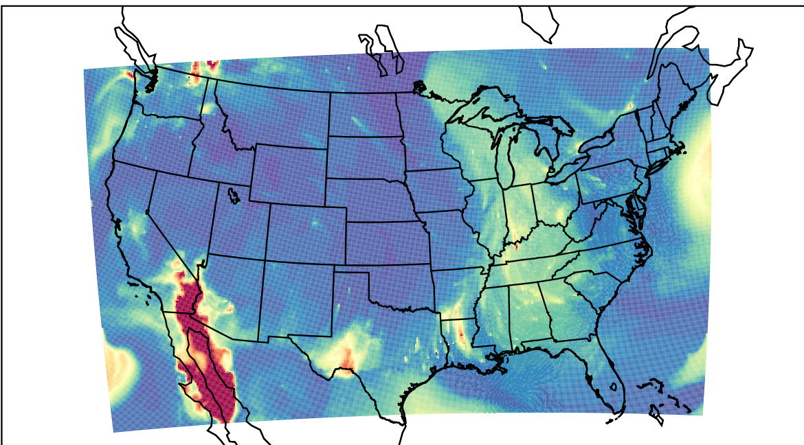
WRF 2019-10-11_10:00:00
