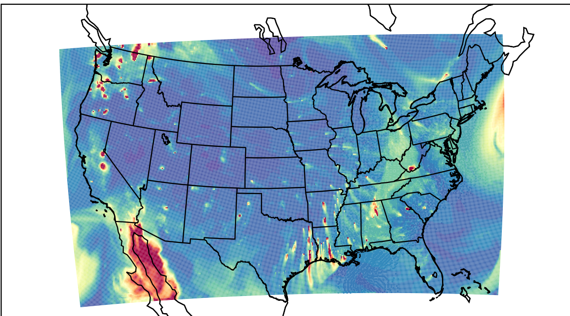
WRF 2019-10-12_02:00:00
