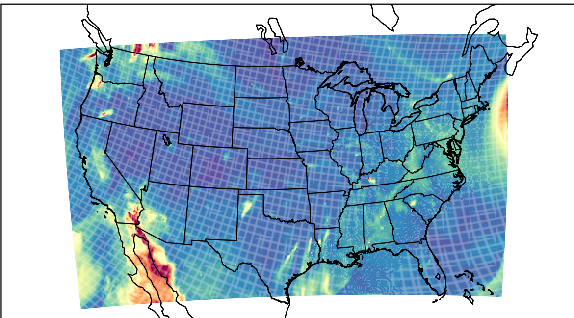
WRF 2019-10-12_09:00:00
