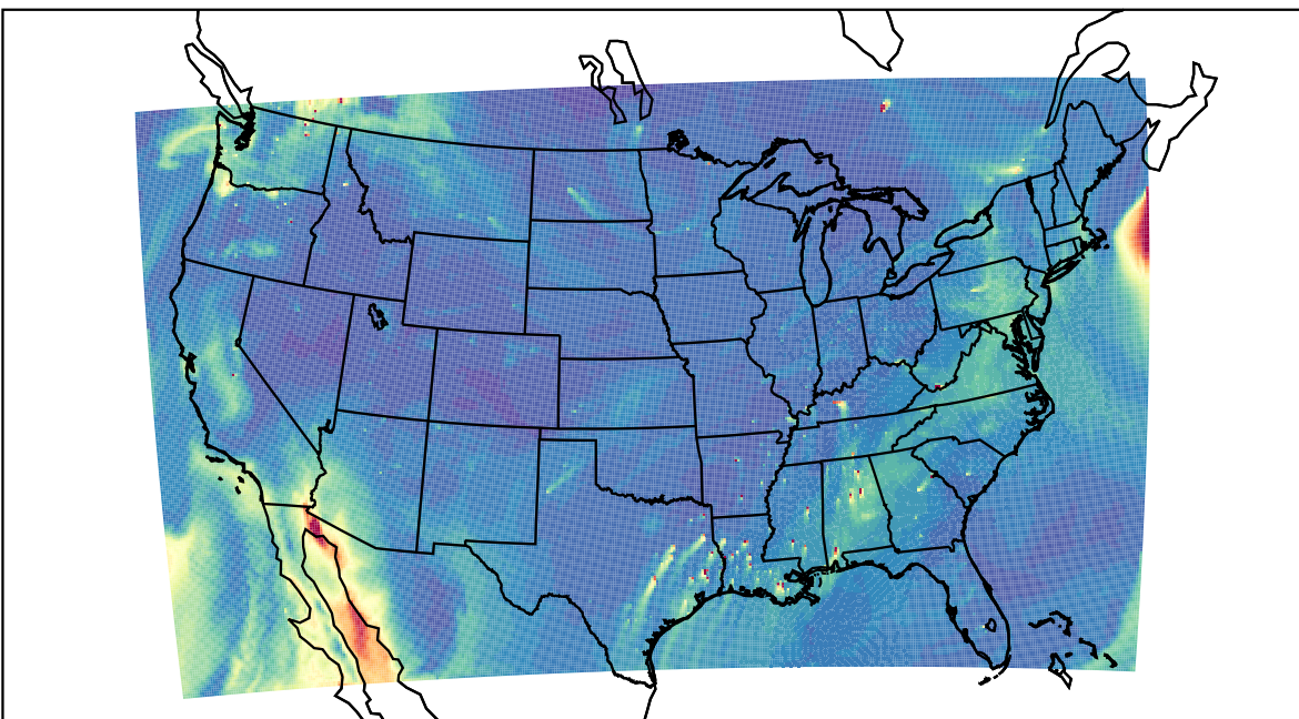
WRF 2019-10-12_19:00:00
