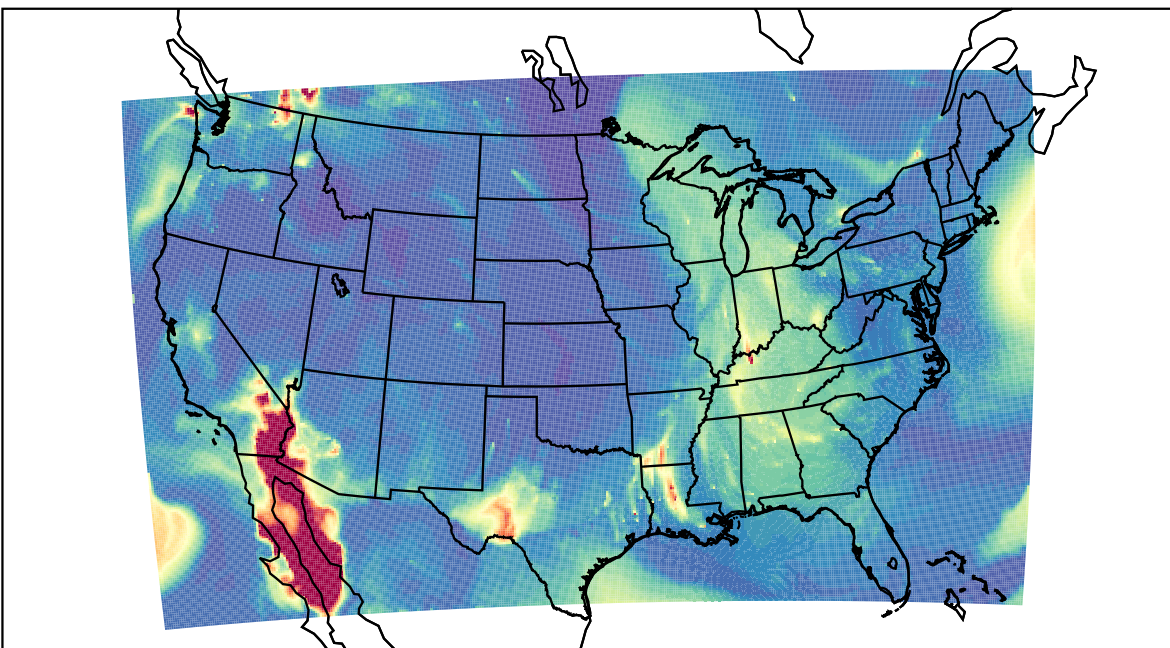
WRF 2019-10-11_09:00:00
