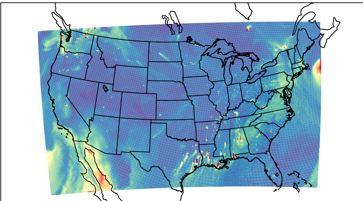
WRF 2019-10-12_22:00:00
