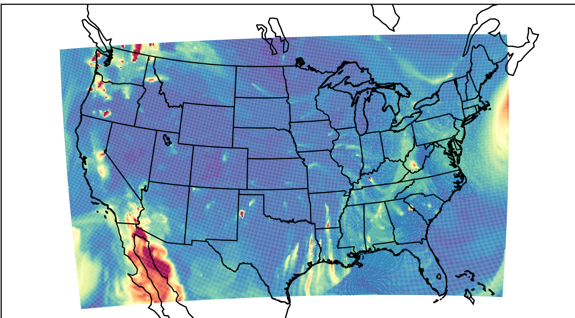
WRF 2019-10-12_05:00:00
