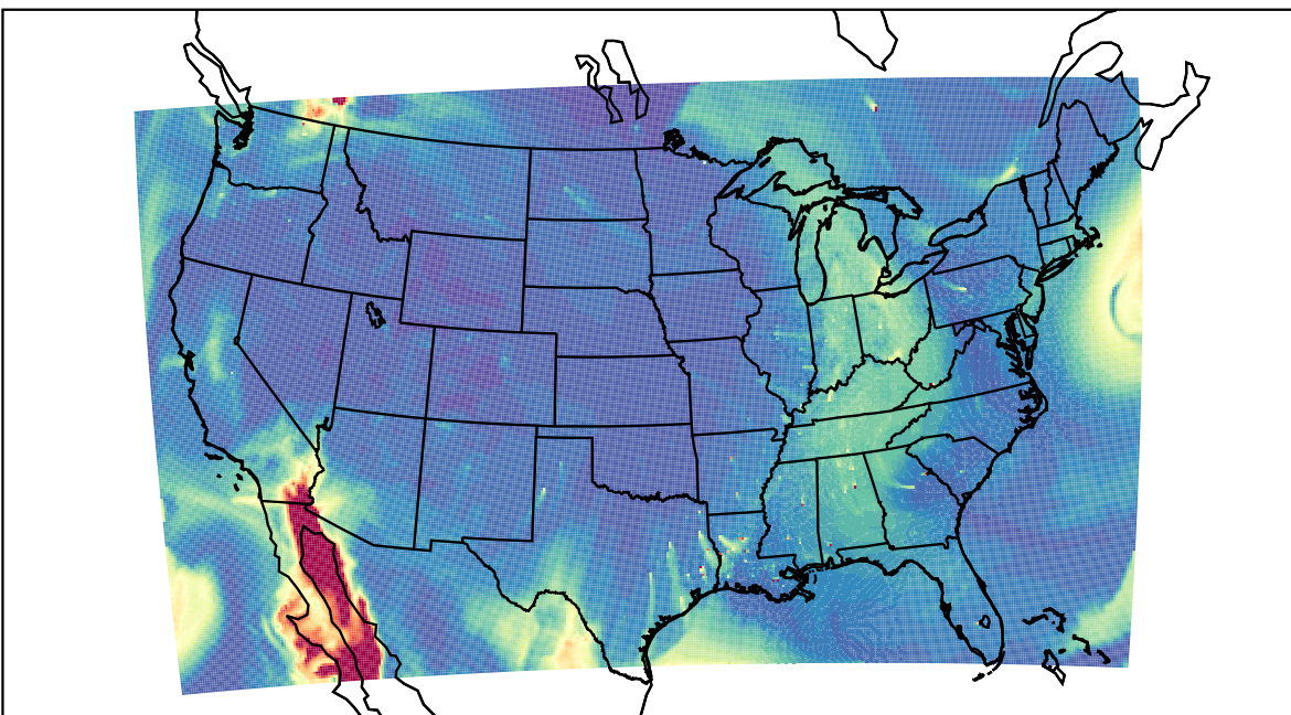
WRF 2019-10-11_18:00:00
