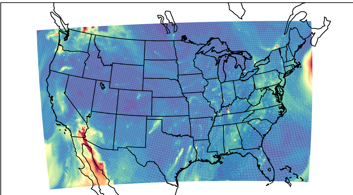
WRF 2019-10-12_13:00:00
