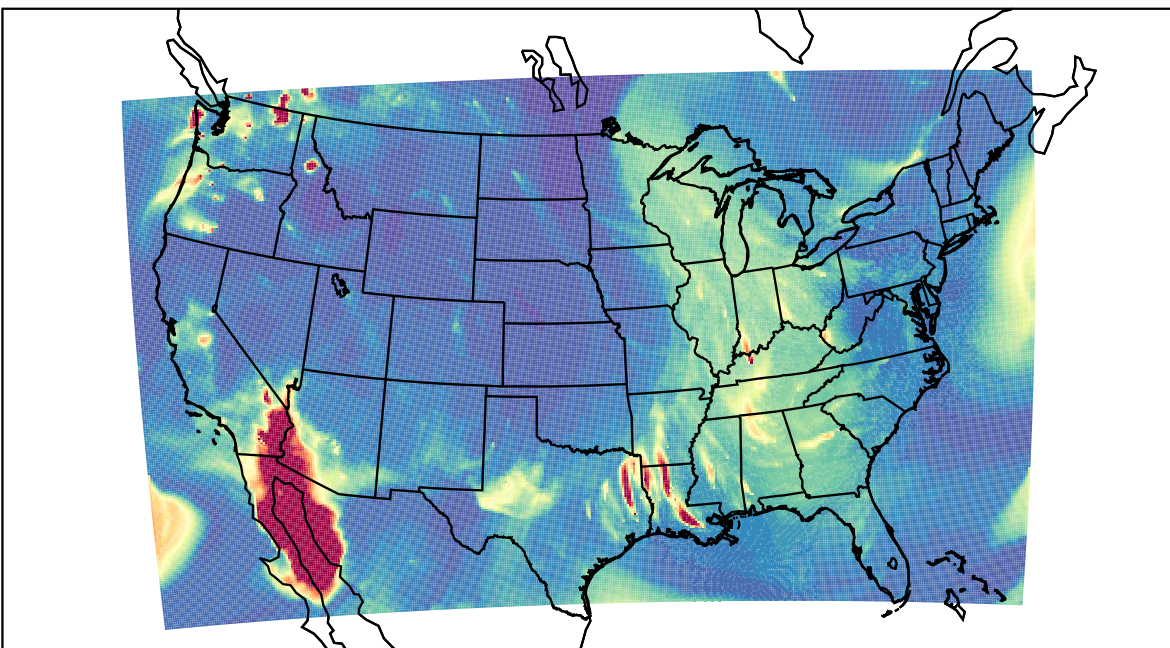
WRF 2019-10-11_05:00:00
