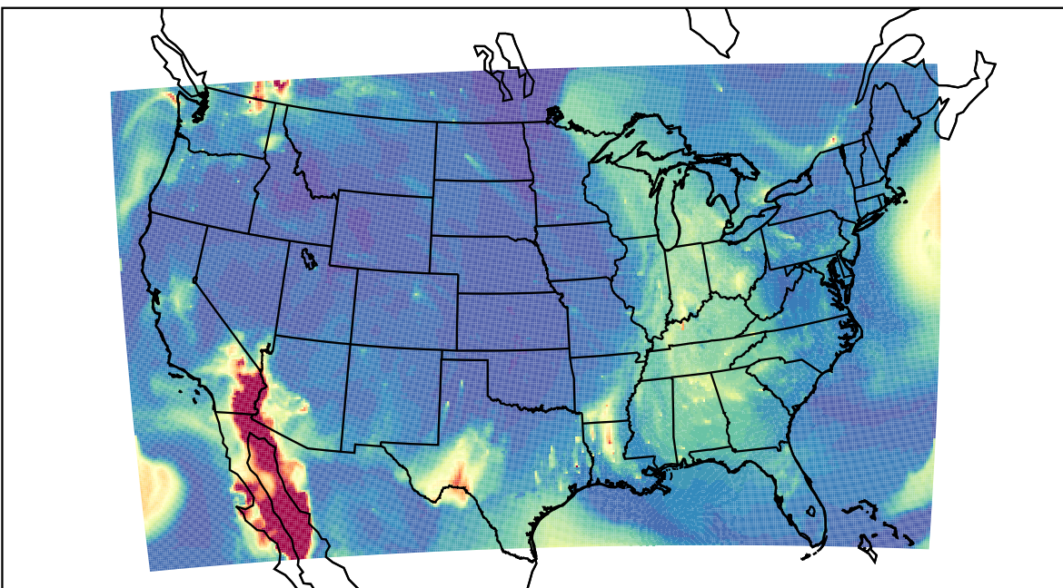
WRF 2019-10-11_11:00:00
