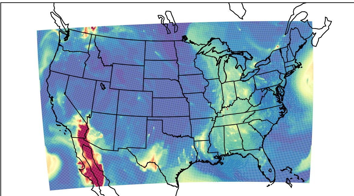
WRF 2019-10-11_12:00:00
