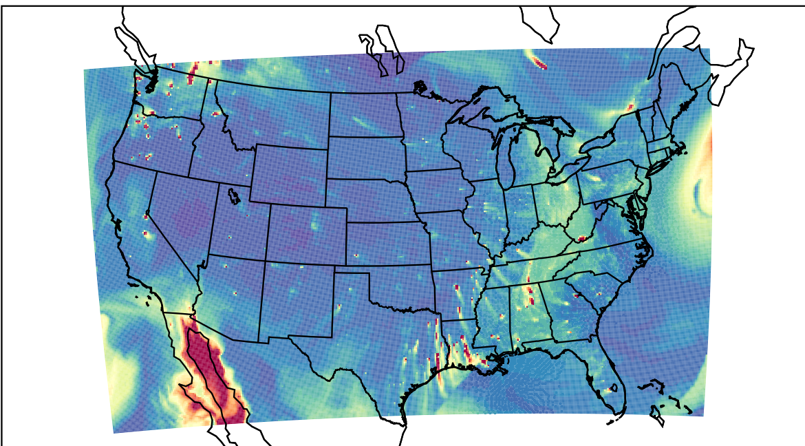
WRF 2019-10-12_00:00:00
