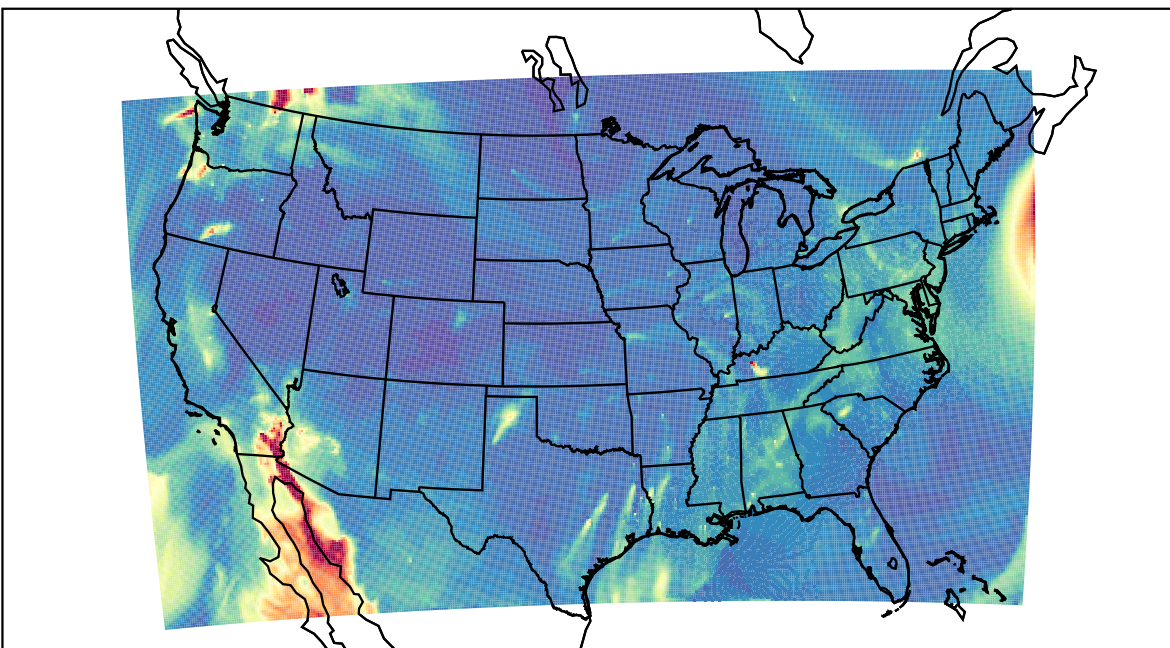
WRF 2019-10-12_10:00:00
