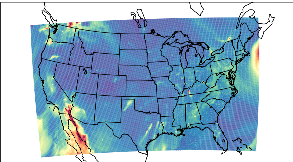
WRF 2019-10-12_12:00:00
