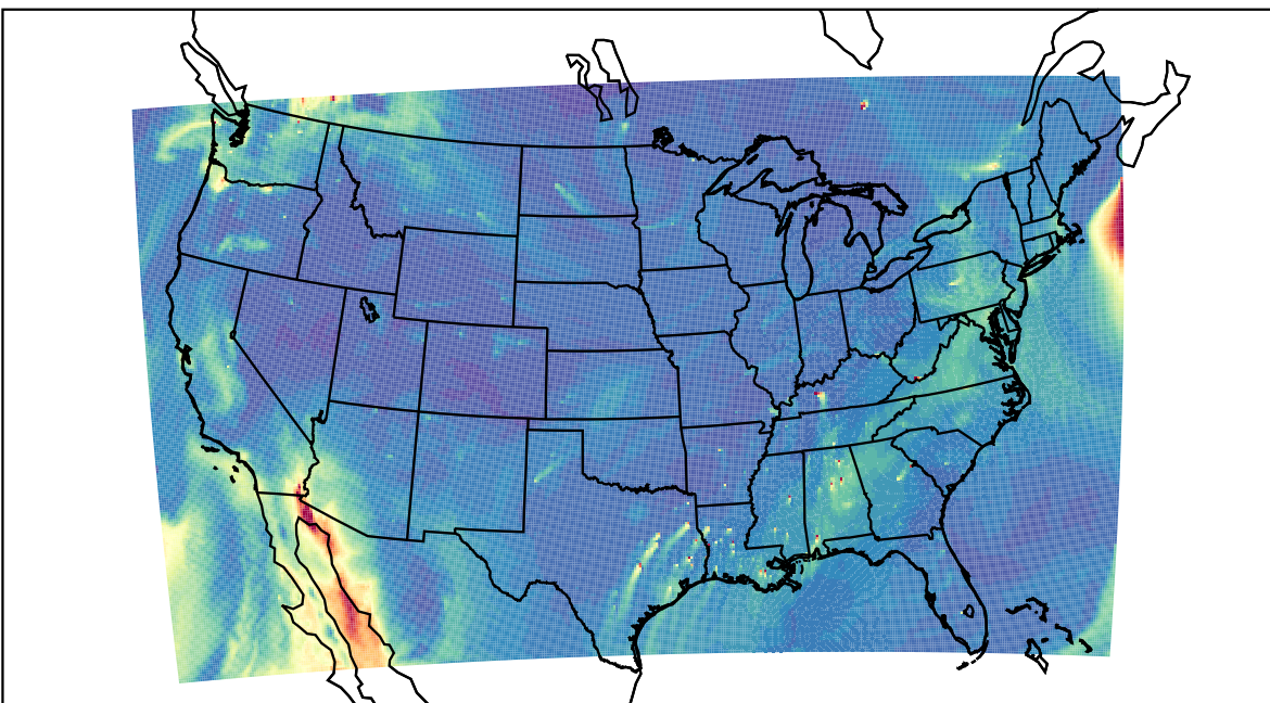
WRF 2019-10-12_18:00:00
