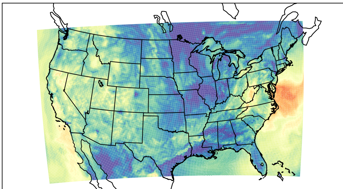
WRF (2019-10-16_08:00:00)
