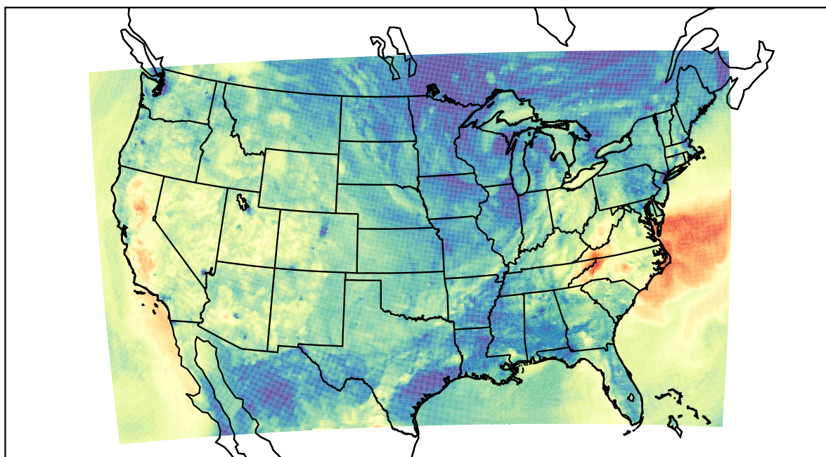
WRF (2019-10-16_02:00:00)
