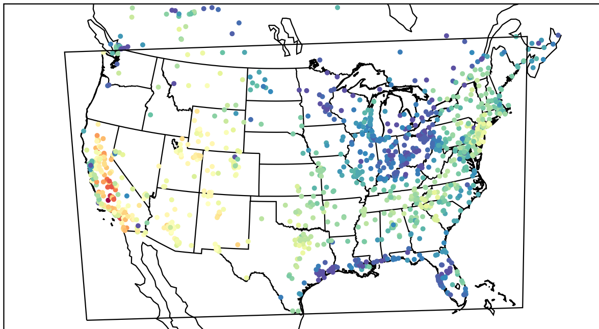
AirNOW (2019-10-16_20:00:00)
