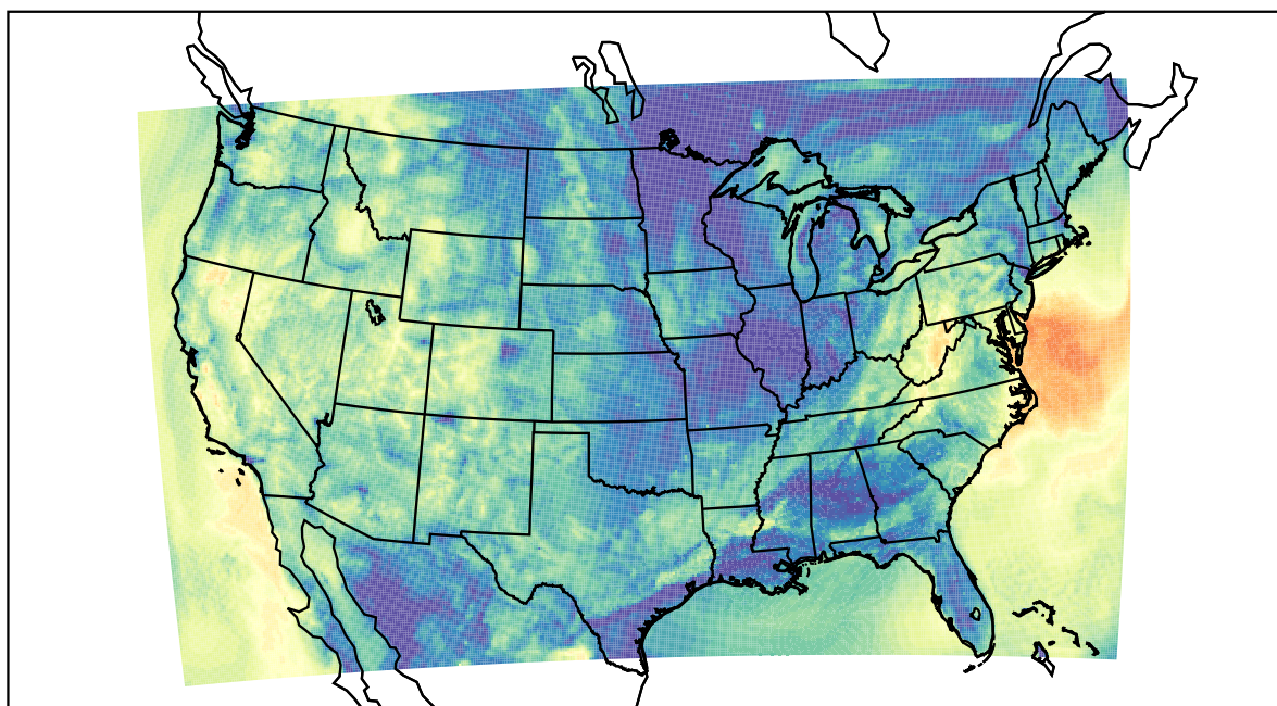
WRF (2019-10-16_09:00:00)
