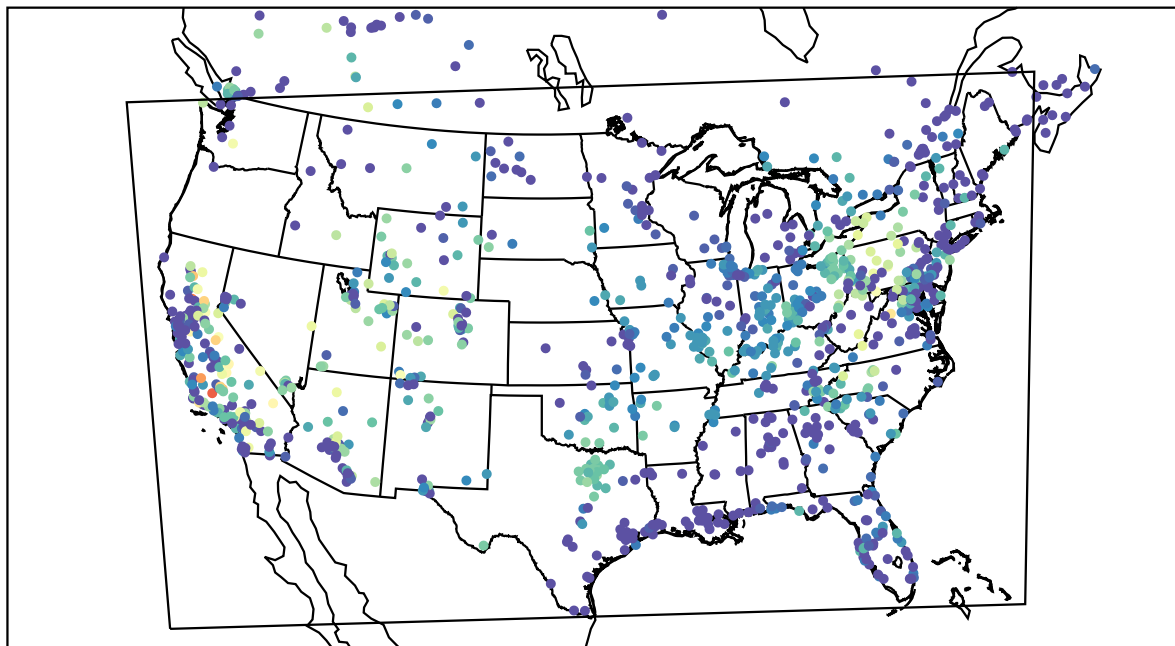
AirNOW (2019-10-16_08:00:00)
