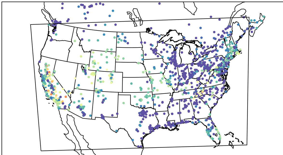
AirNOW (2019-10-15_03:00:00)
