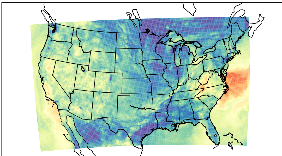
WRF (2019-10-16_04:00:00)
