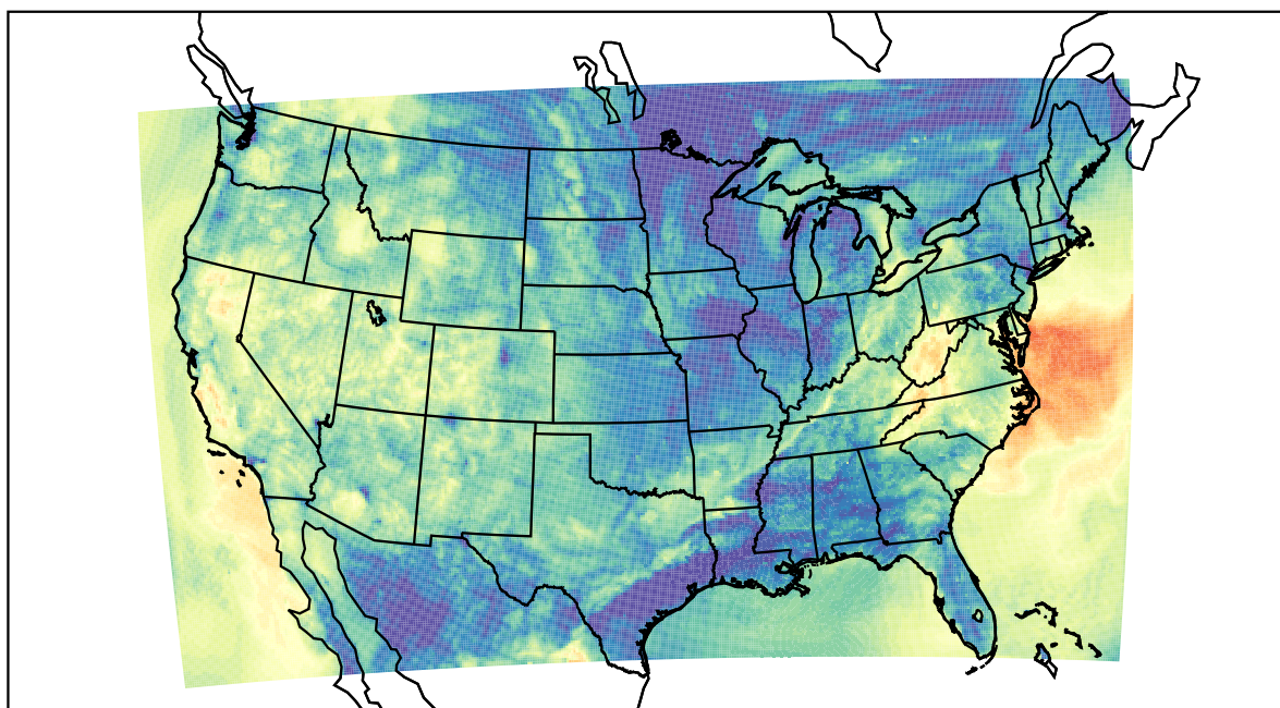
WRF (2019-10-16_06:00:00)
