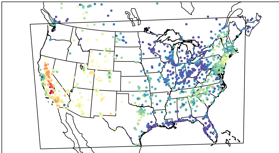
AirNOW (2019-10-16_23:00:00)
