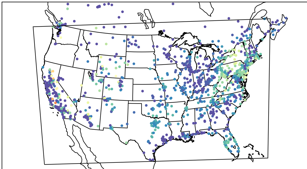
AirNOW (2019-10-16_14:00:00)
