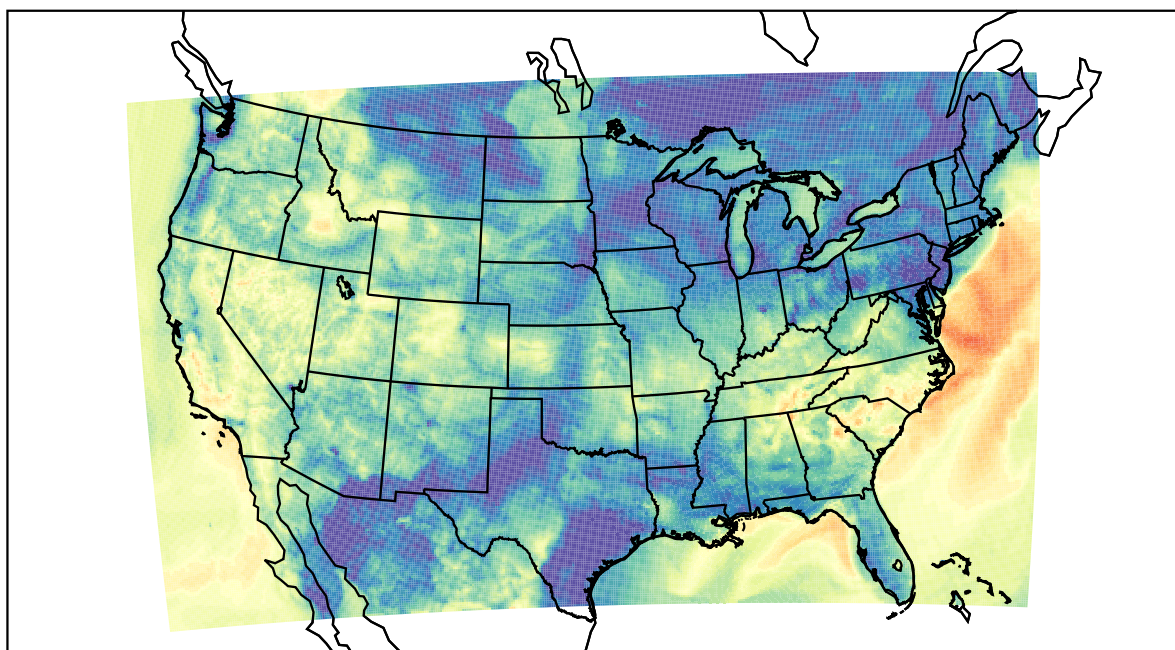
WRF (2019-10-15_06:00:00)
