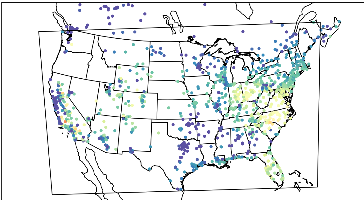
AirNOW (2019-10-15_16:00:00)
