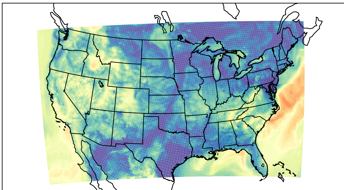
WRF (2019-10-15_10:00:00)
