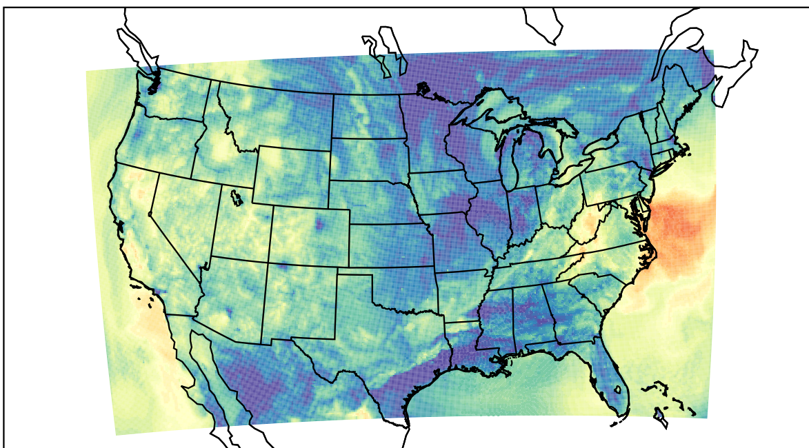
WRF (2019-10-16_07:00:00)
