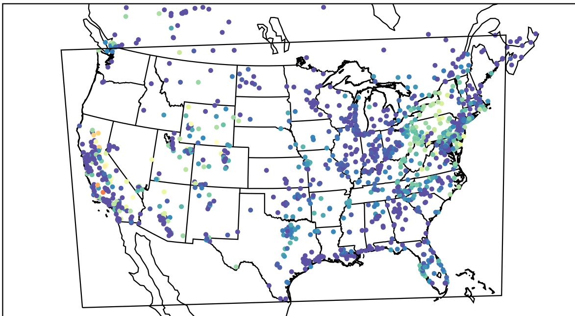
AirNOW (2019-10-16_13:00:00)
