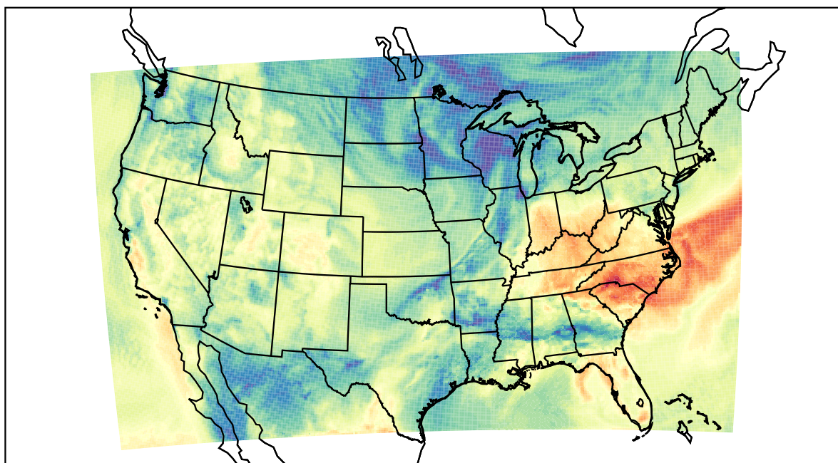
WRF (2019-10-15_18:00:00)
