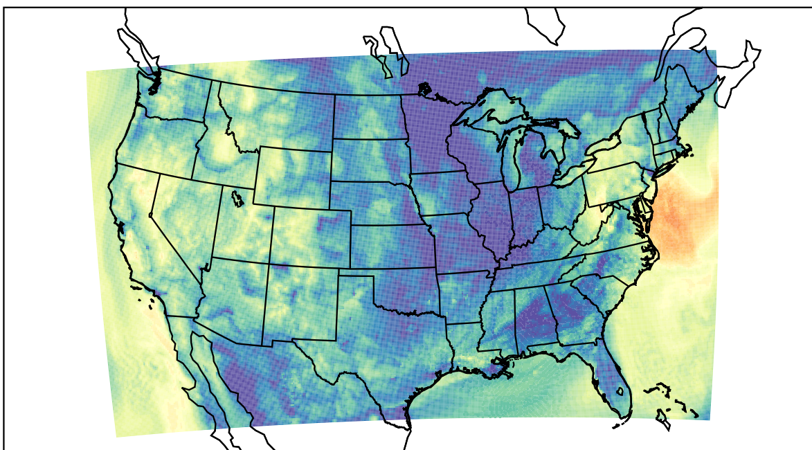
WRF (2019-10-16_13:00:00)
