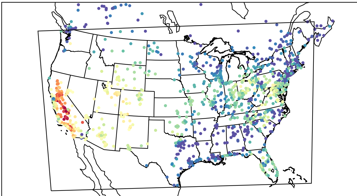
AirNOW (2019-10-15_23:00:00)
