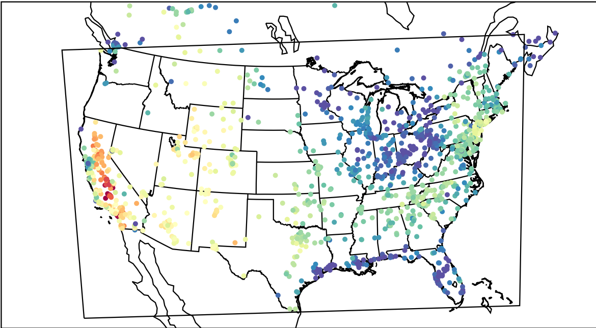
AirNOW (2019-10-16_22:00:00)
