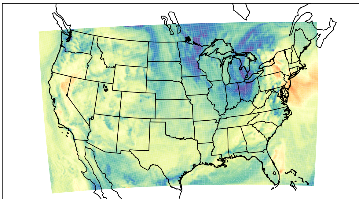
WRF (2019-10-16_18:00:00)
