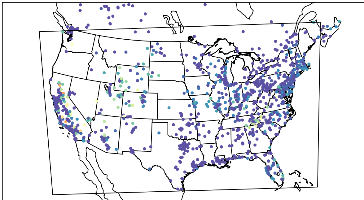
AirNOW (2019-10-15_13:00:00)
