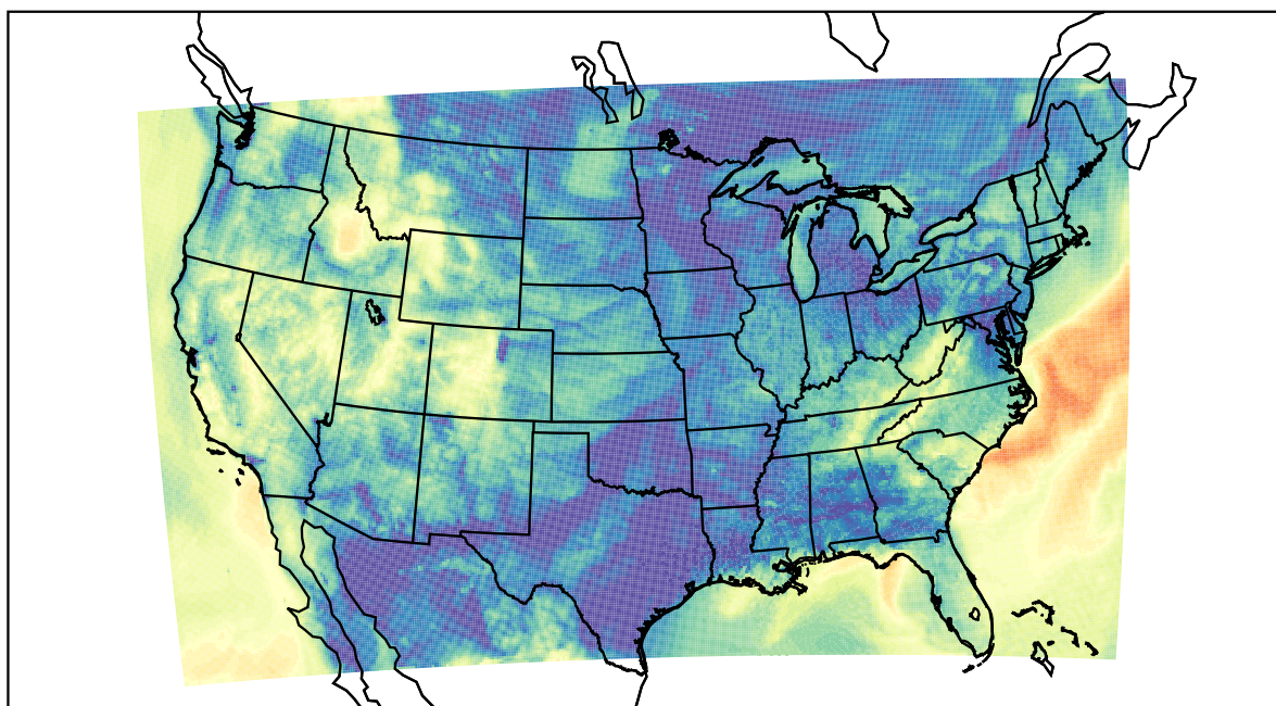
WRF (2019-10-15_14:00:00)
