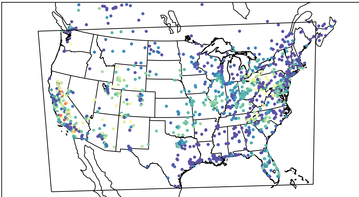
AirNOW (2019-10-16_03:00:00)
