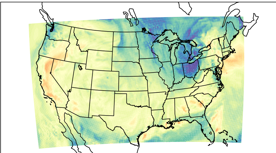
WRF (2019-10-16_21:00:00)
