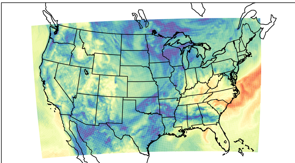
WRF (2019-10-15_16:00:00)
