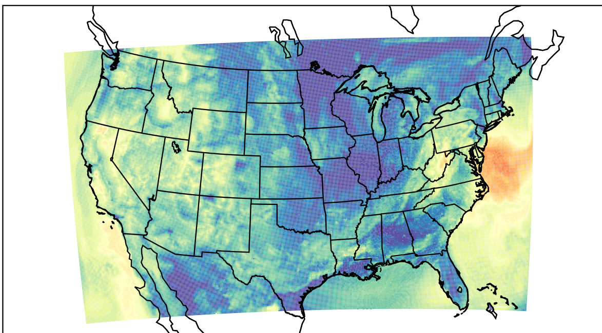
WRF (2019-10-16_10:00:00)
