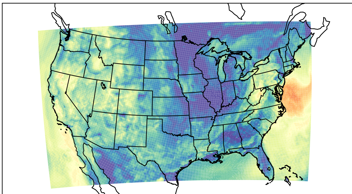
WRF (2019-10-16_11:00:00)
