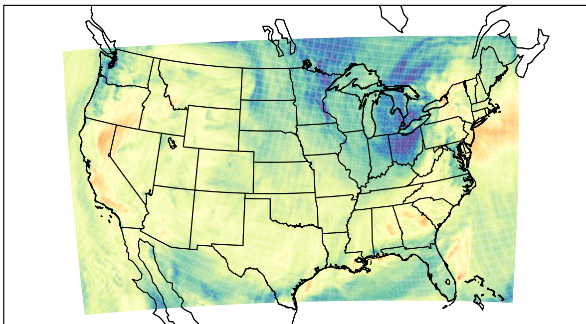
WRF (2019-10-16_20:00:00)
