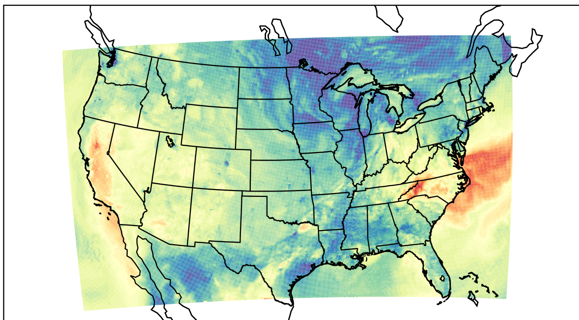
WRF (2019-10-16_00:00:00)
