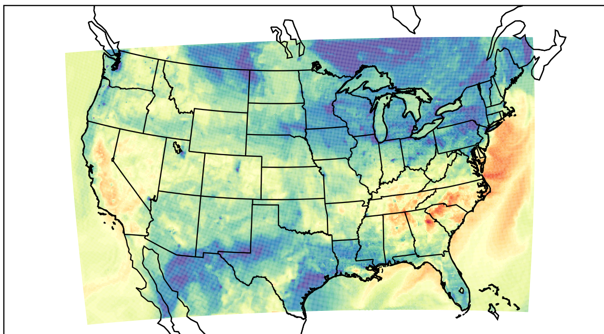
WRF (2019-10-15_01:00:00)
