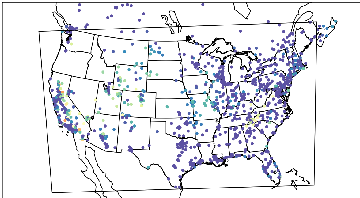
AirNOW (2019-10-15_10:00:00)
