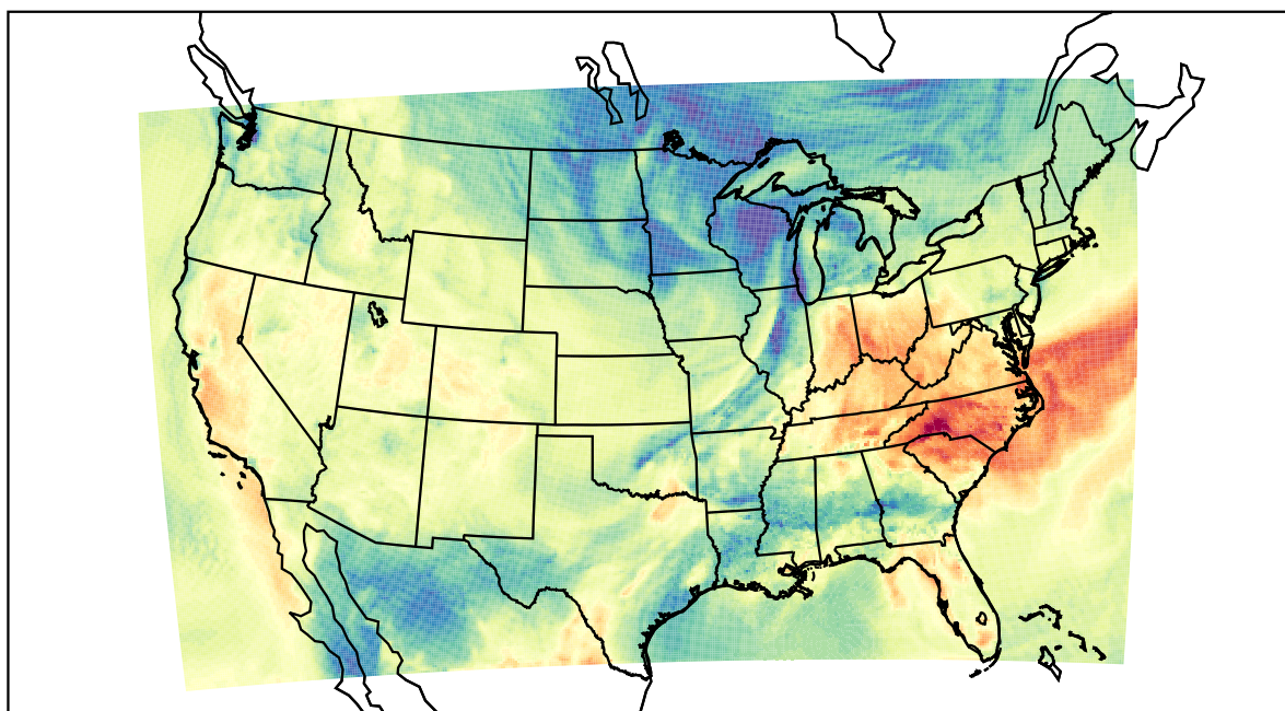
WRF (2019-10-15_20:00:00)
