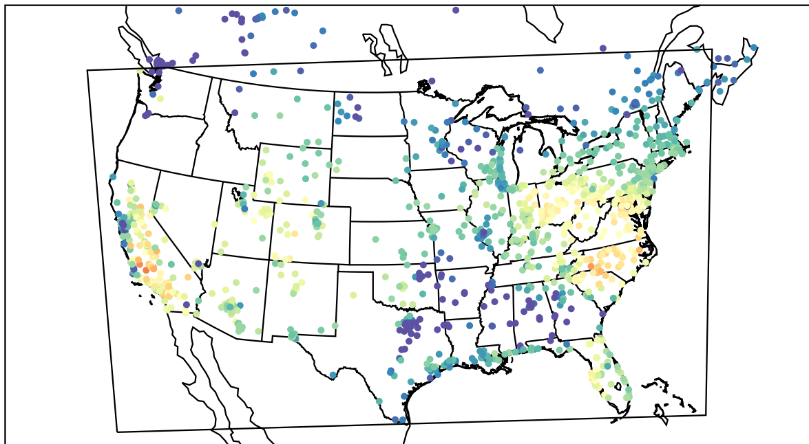
AirNOW (2019-10-15_18:00:00)
