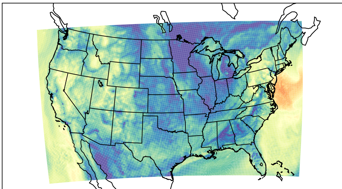
WRF (2019-10-16_14:00:00)
