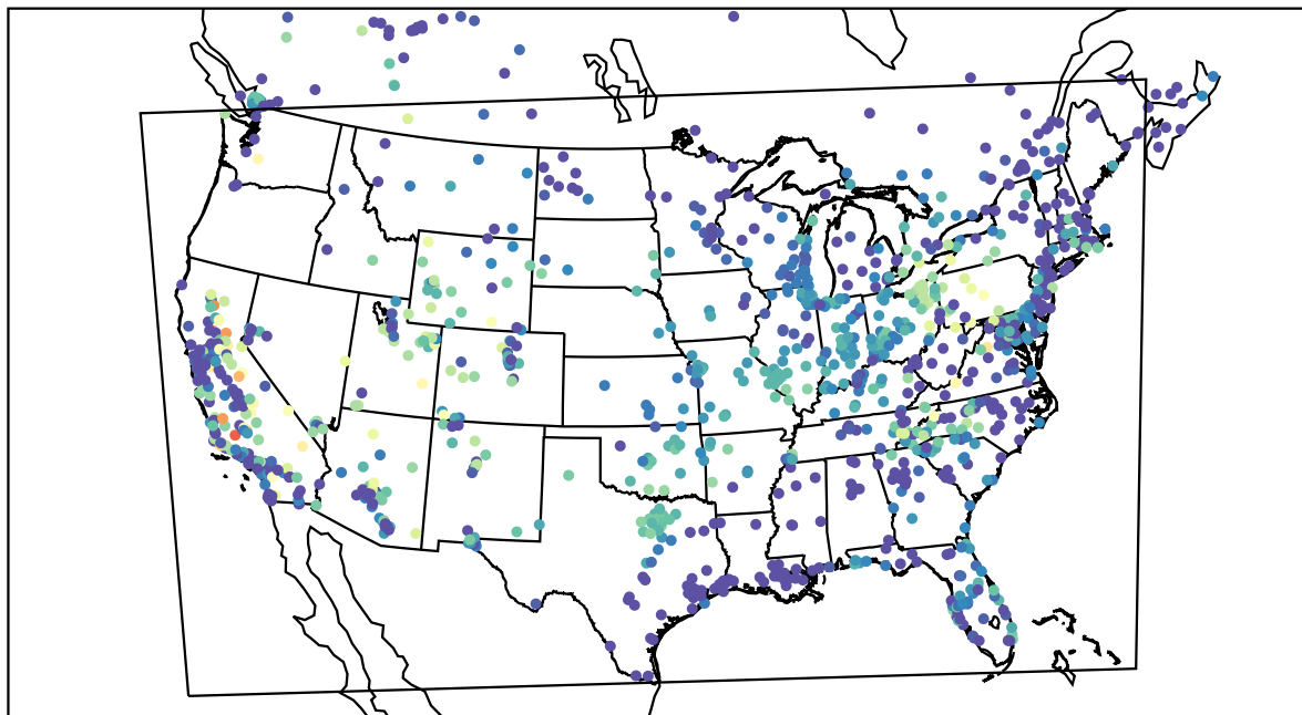
AirNOW (2019-10-16_06:00:00)
