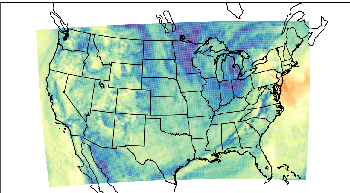
WRF (2019-10-16_16:00:00)
