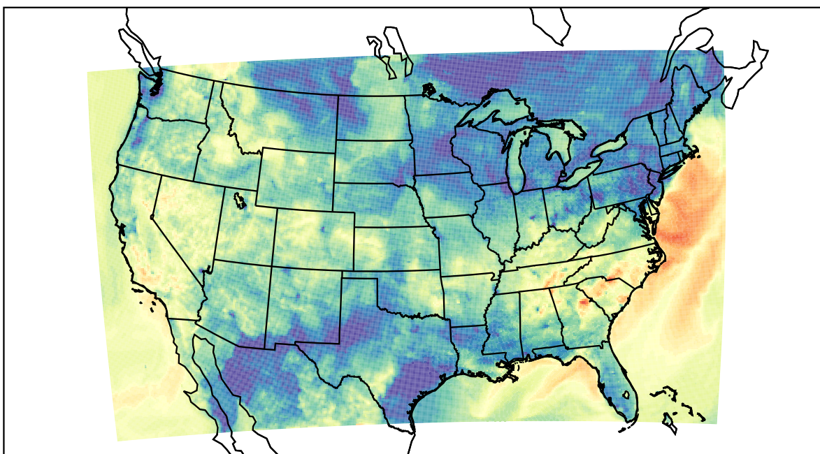
WRF (2019-10-15_04:00:00)
