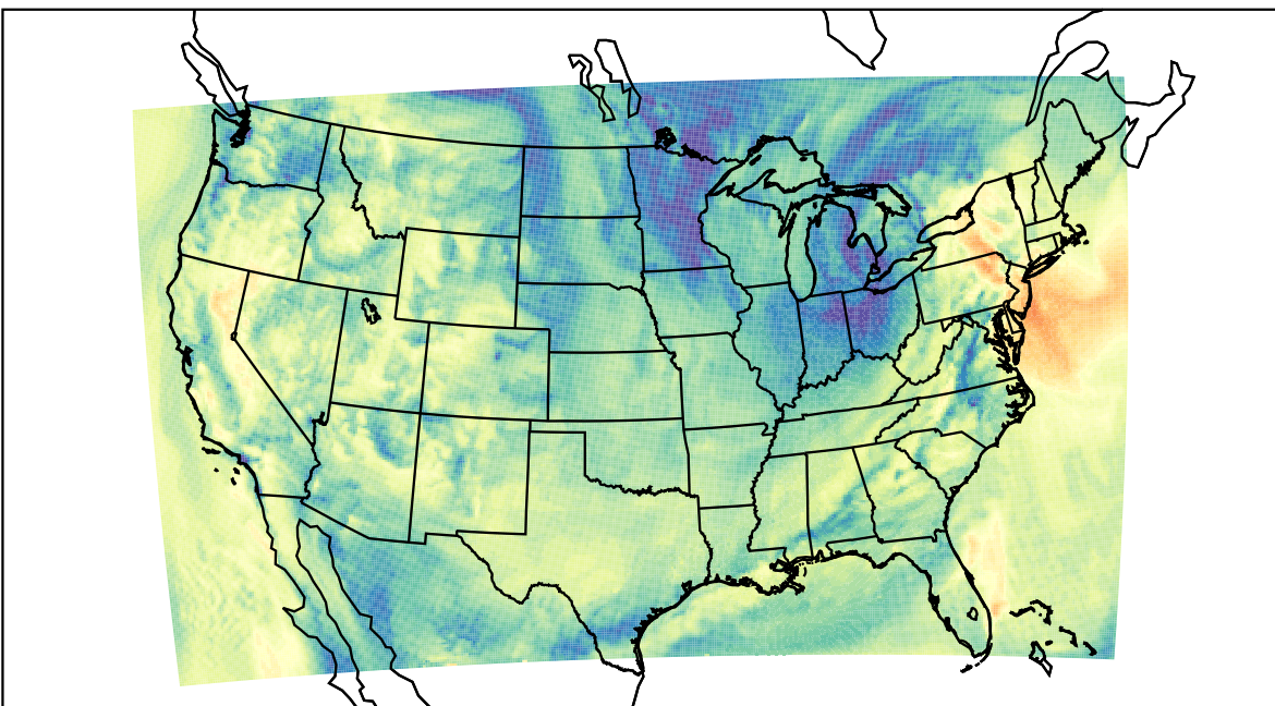
WRF (2019-10-16_17:00:00)
