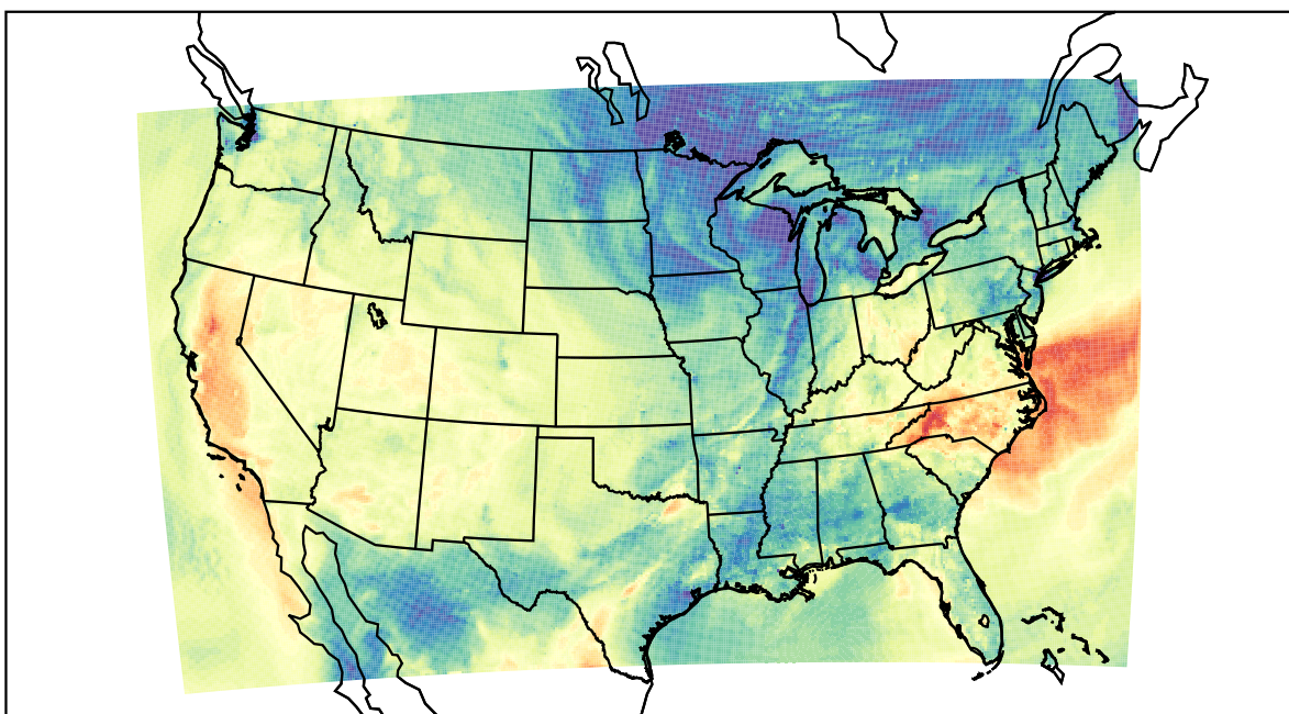
WRF (2019-10-15_23:00:00)
