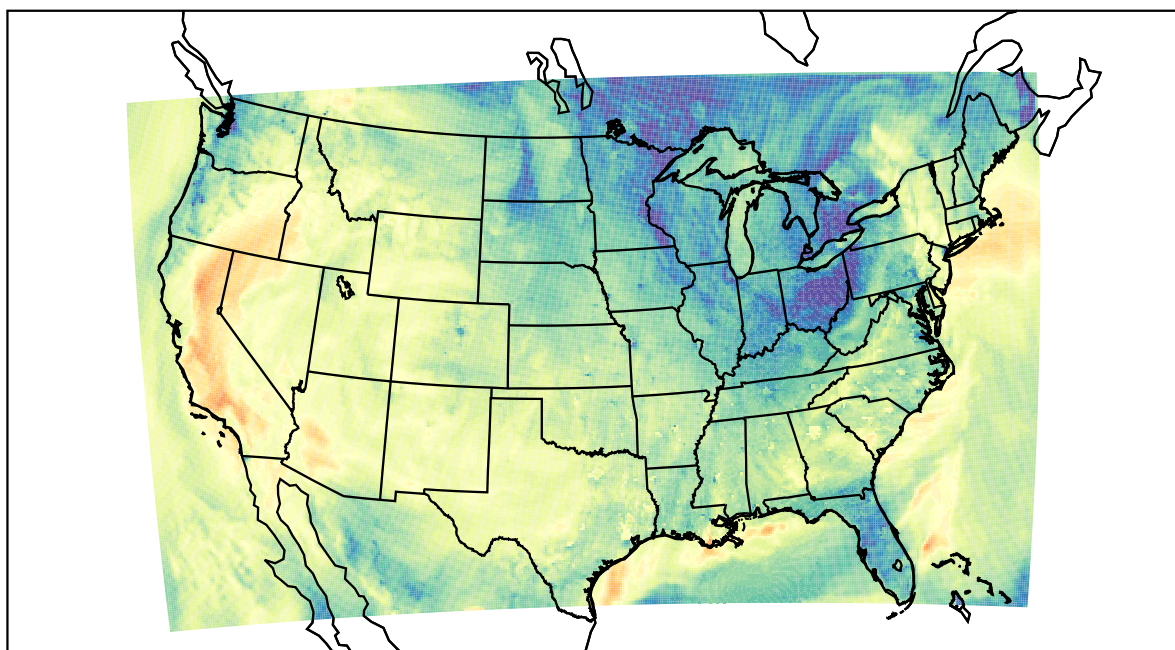
WRF (2019-10-16_23:00:00)
