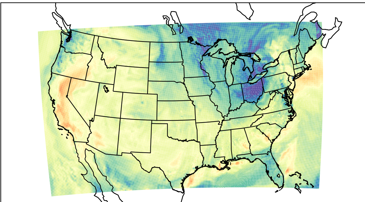
WRF (2019-10-16_22:00:00)
