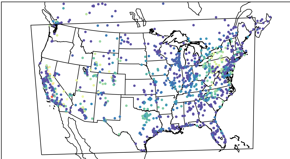
AirNOW (2019-10-16_10:00:00)
