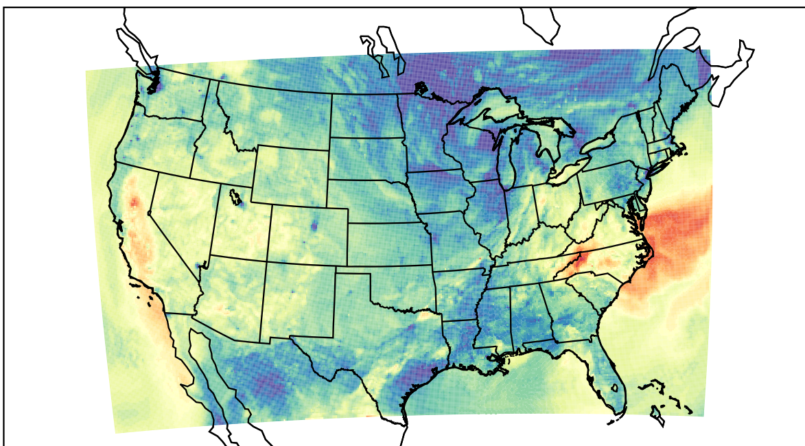
WRF (2019-10-16_01:00:00)
