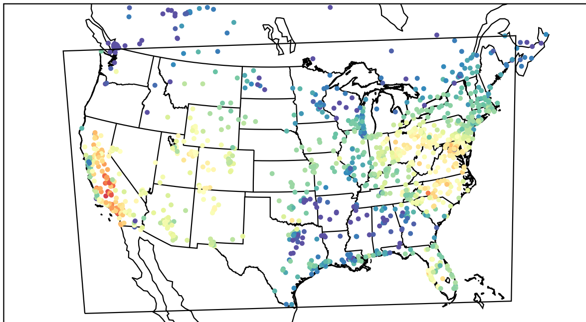
AirNOW (2019-10-15_20:00:00)
