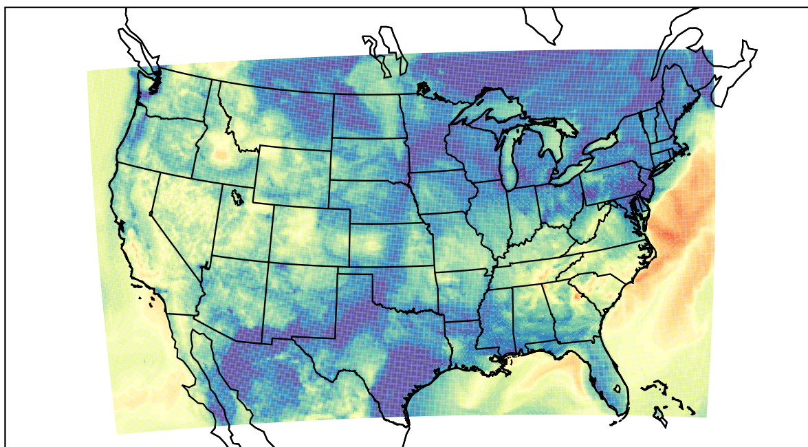
WRF (2019-10-15_07:00:00)
