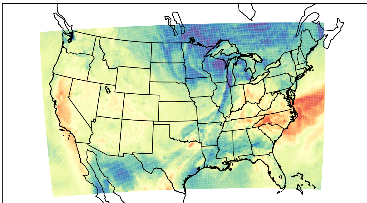
WRF (2019-10-15_22:00:00)
