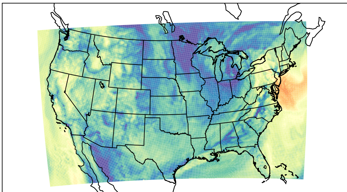
WRF (2019-10-16_15:00:00)
