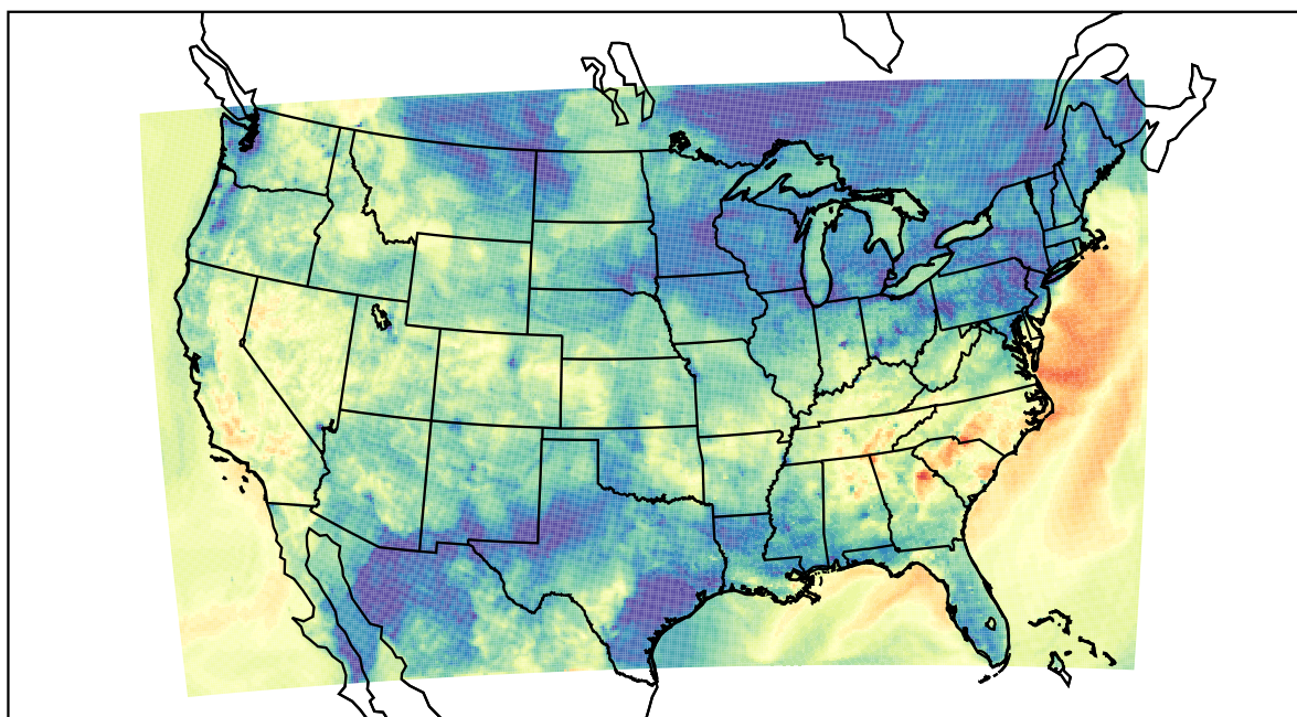
WRF (2019-10-15_03:00:00)
