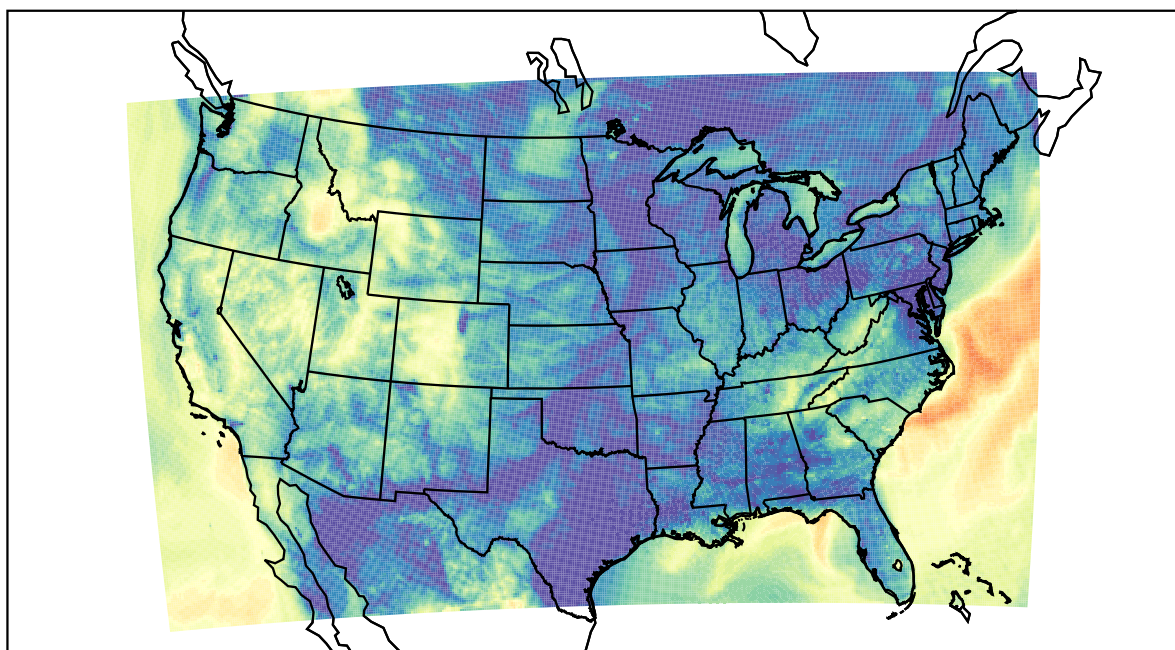
WRF (2019-10-15_13:00:00)
