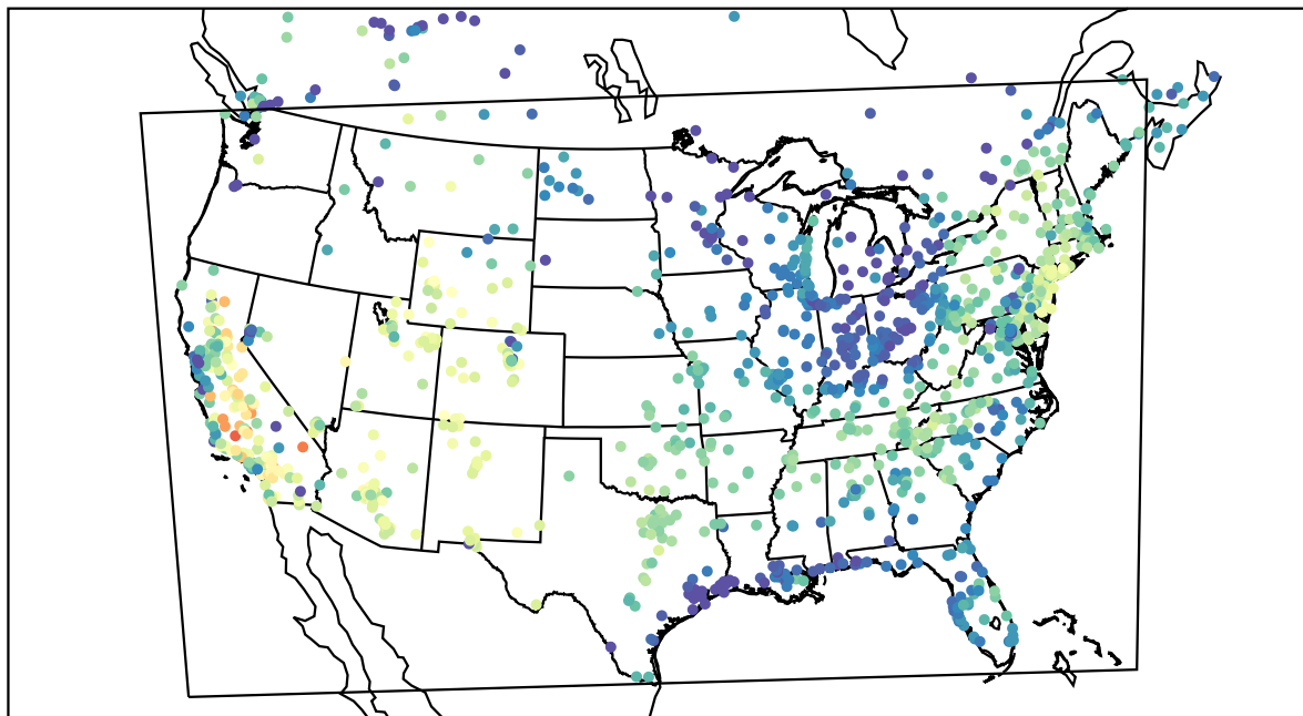
AirNOW (2019-10-16_18:00:00)
