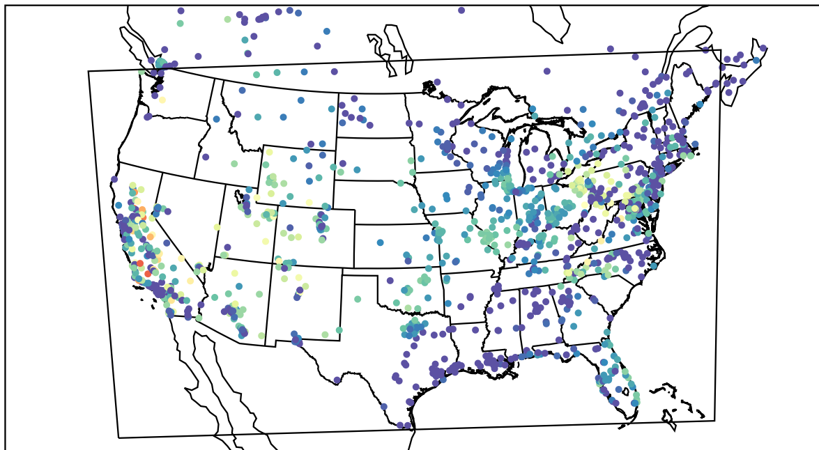
AirNOW (2019-10-16_04:00:00)
