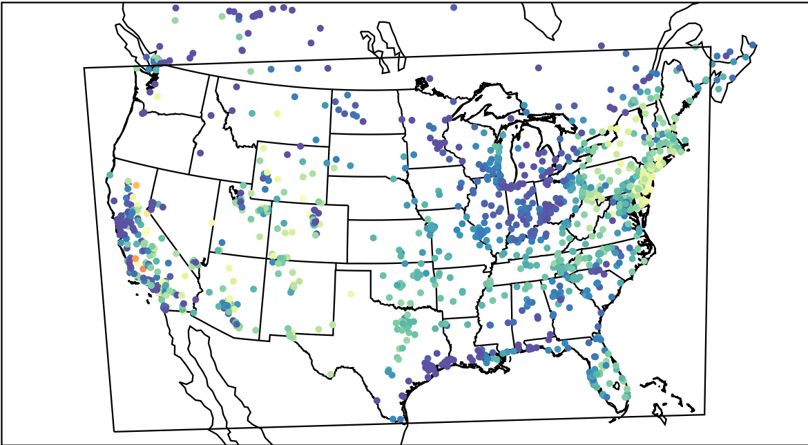
AirNOW (2019-10-16_16:00:00)
