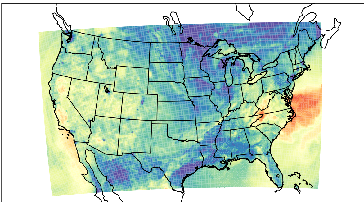
WRF (2019-10-16_03:00:00)
