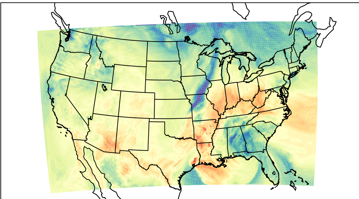
WRF (2019-10-19_20:00:00)
