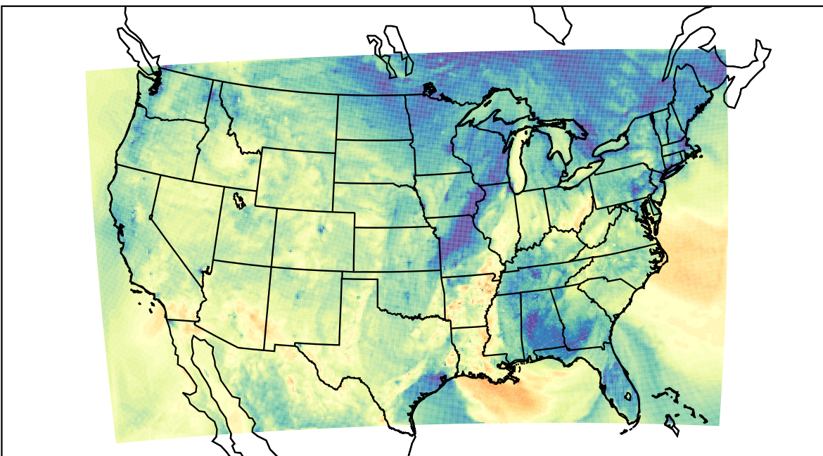
WRF (2019-10-20_01:00:00)
