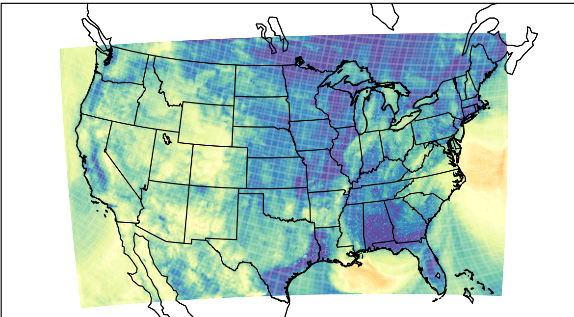
WRF (2019-10-20_10:00:00)
