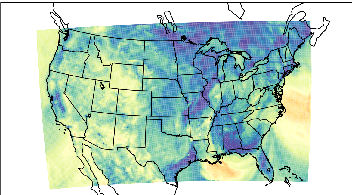
WRF (2019-10-20_07:00:00)
