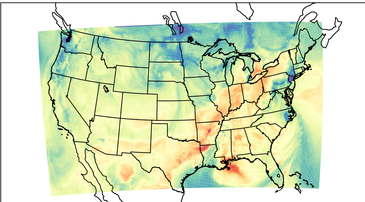
WRF (2019-10-20_19:00:00)
