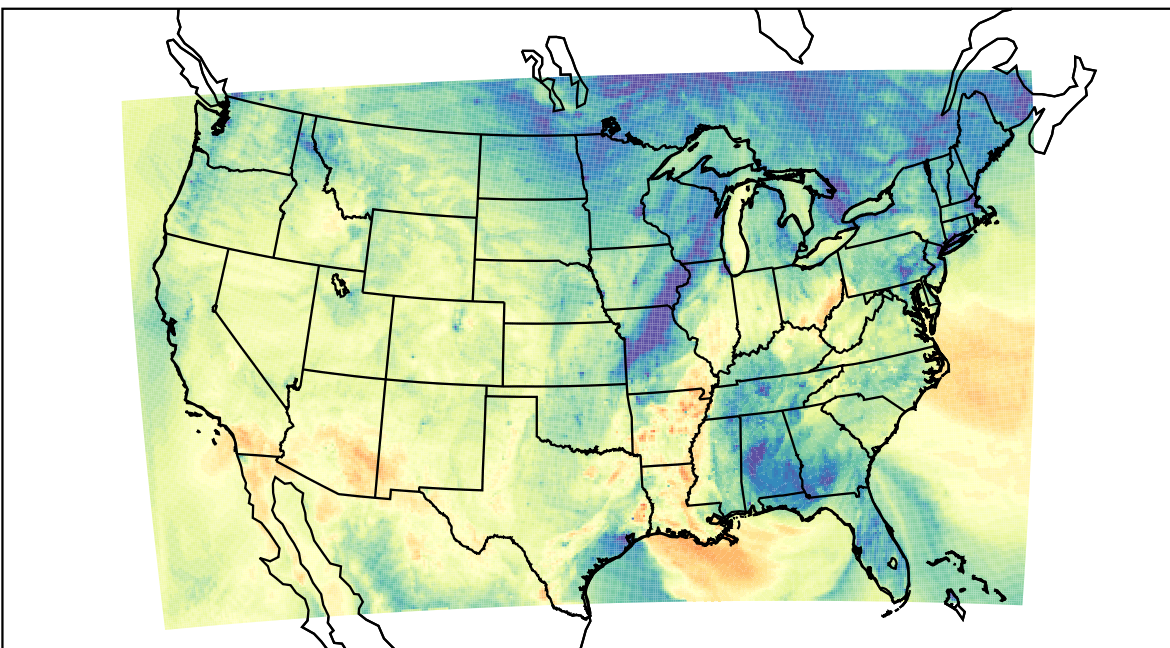
WRF (2019-10-20_00:00:00)
