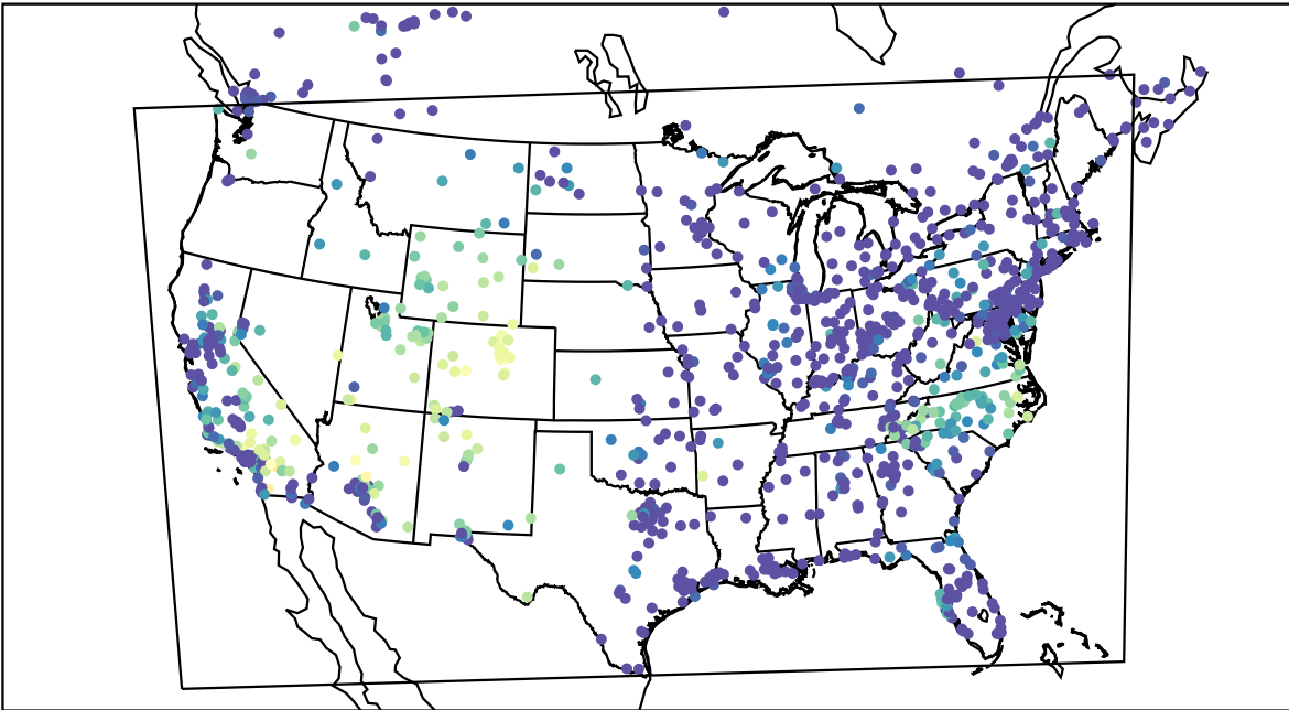
AirNOW (2019-10-20_11:00:00)
