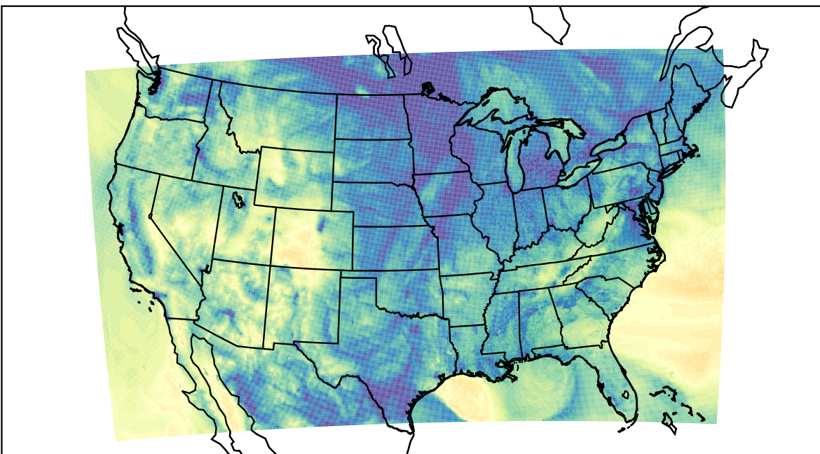
WRF (2019-10-19_14:00:00)
