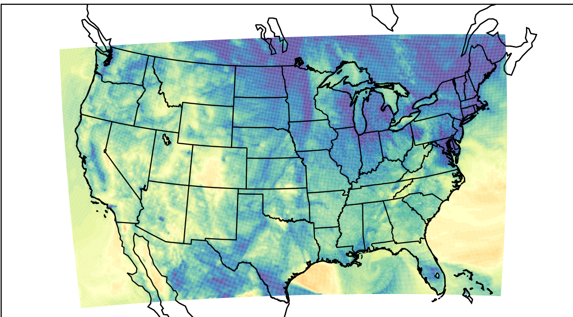
WRF (2019-10-19_08:00:00)
