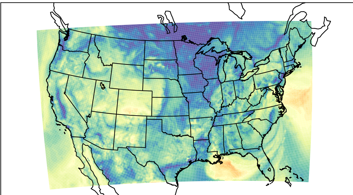
WRF (2019-10-20_15:00:00)
