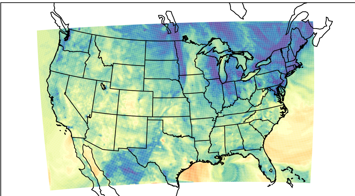
WRF (2019-10-19_03:00:00)
