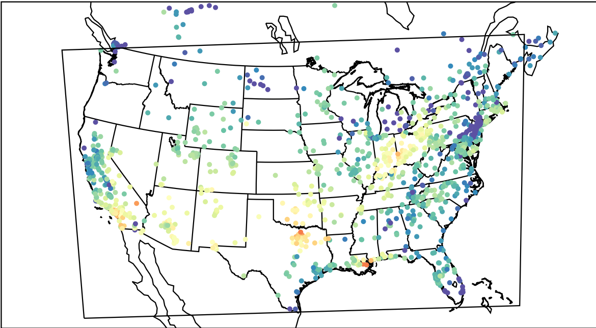
AirNOW (2019-10-20_18:00:00)
