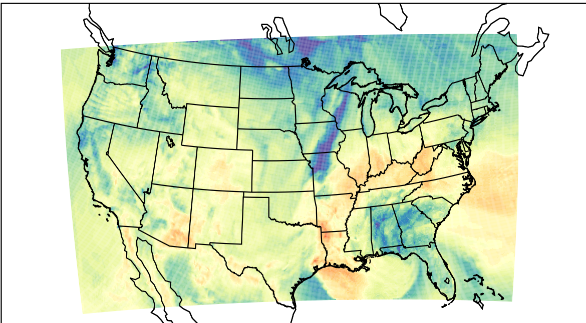
WRF (2019-10-19_18:00:00)
