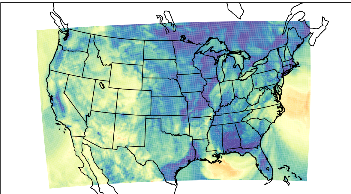
WRF (2019-10-20_09:00:00)
