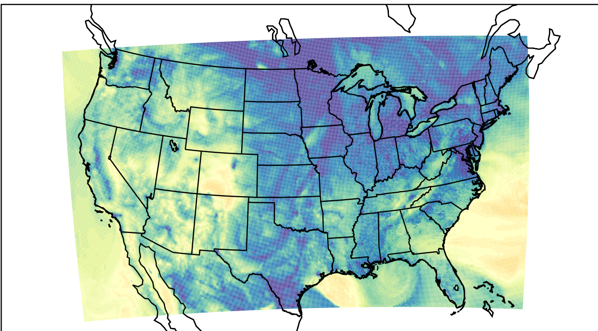
WRF (2019-10-19_13:00:00)
