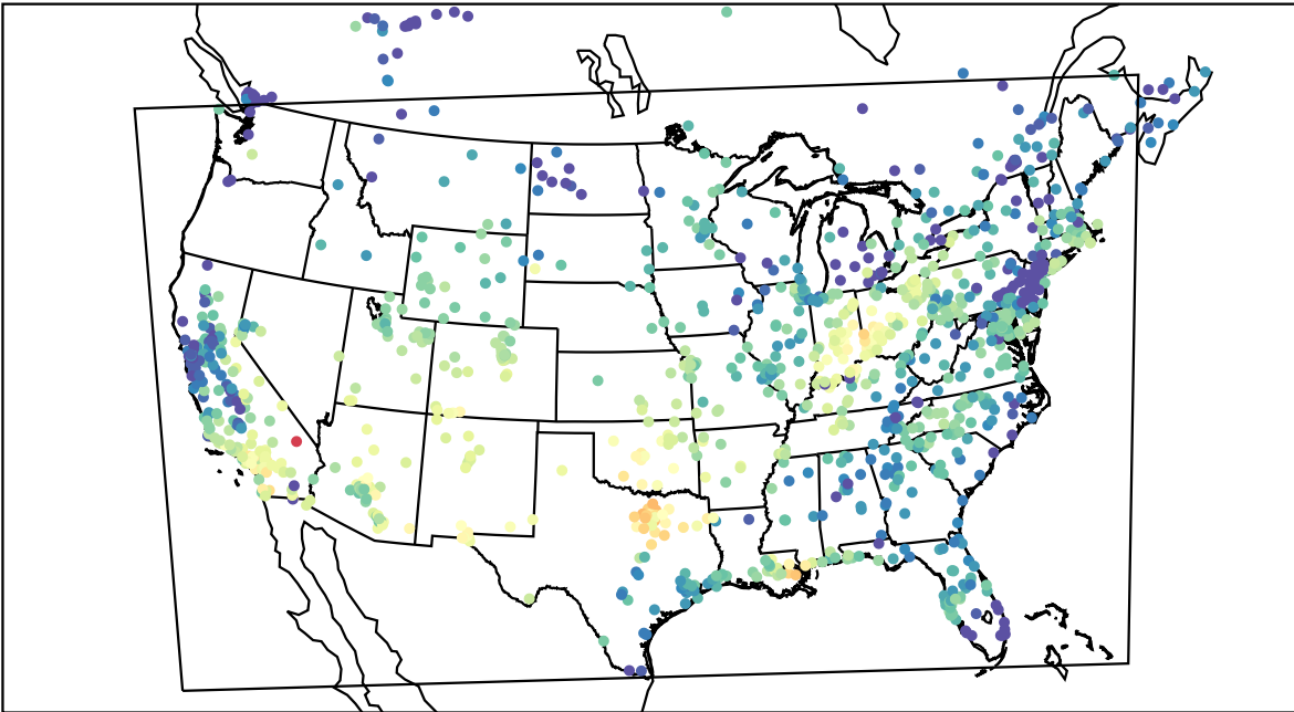
AirNOW (2019-10-20_17:00:00)
