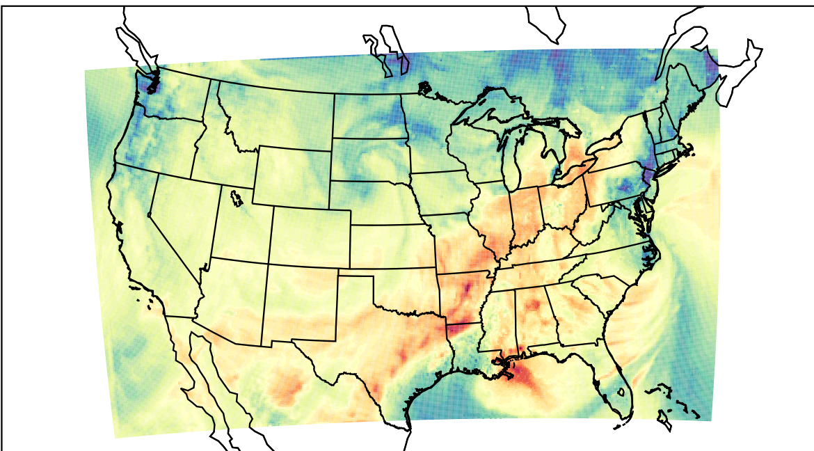
WRF (2019-10-20_21:00:00)
