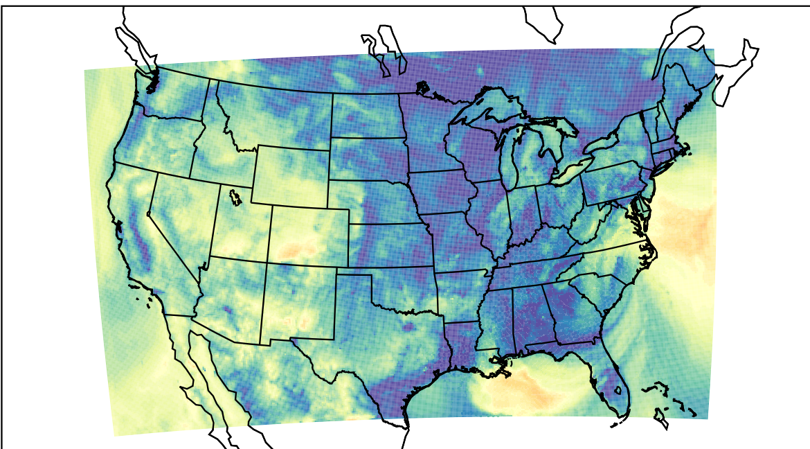
WRF (2019-10-20_13:00:00)
