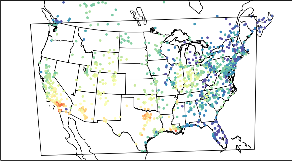
AirNOW (2019-10-19_22:00:00)
