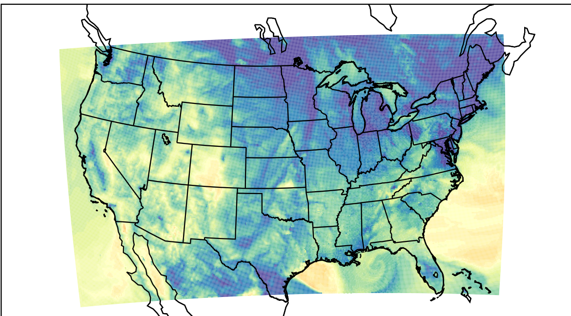
WRF (2019-10-19_10:00:00)
