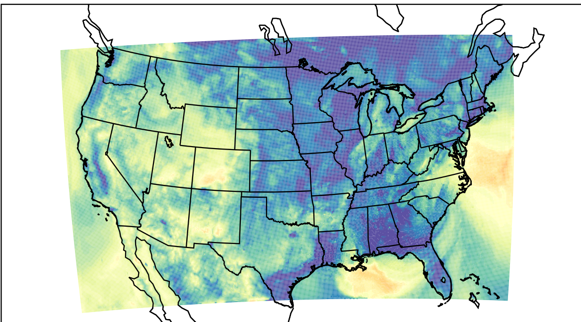
WRF (2019-10-20_12:00:00)
