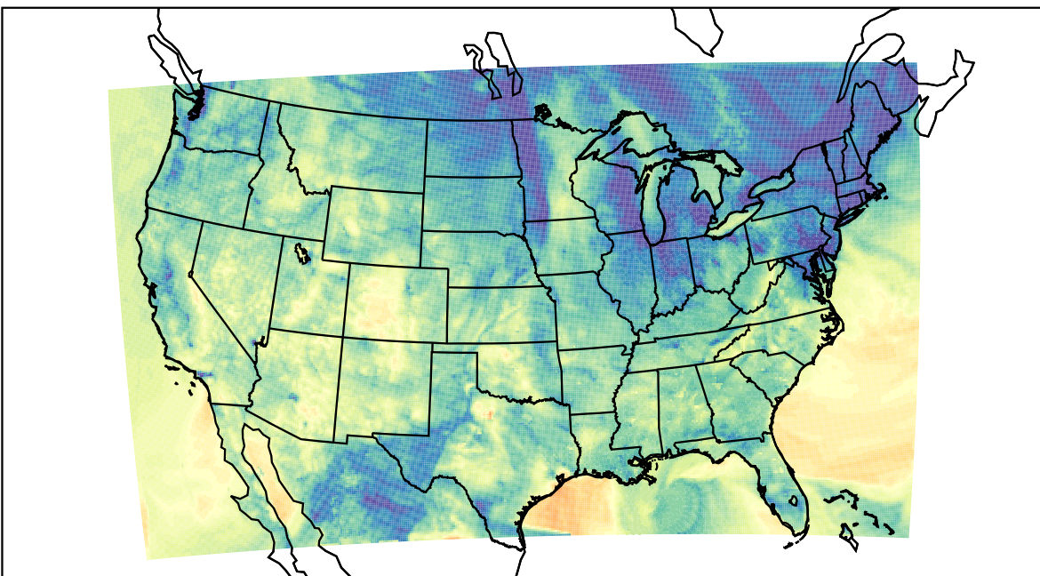
WRF (2019-10-19_04:00:00)
