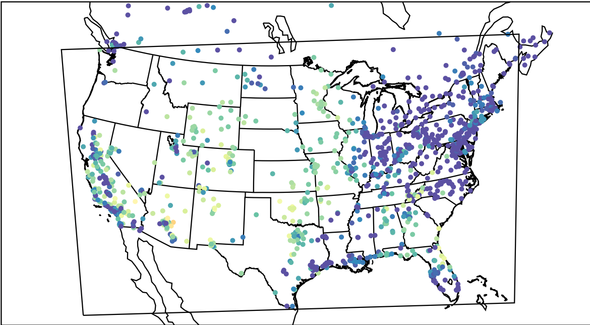
AirNOW (2019-10-19_04:00:00)
