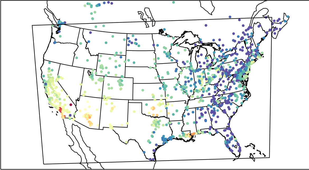
AirNOW (2019-10-20_23:00:00)
