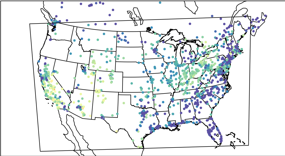
AirNOW (2019-10-22_01:00:00)
