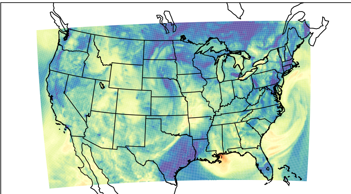
WRF (2019-10-21_06:00:00)
