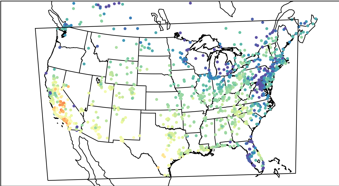
AirNOW (2019-10-22_20:00:00)
