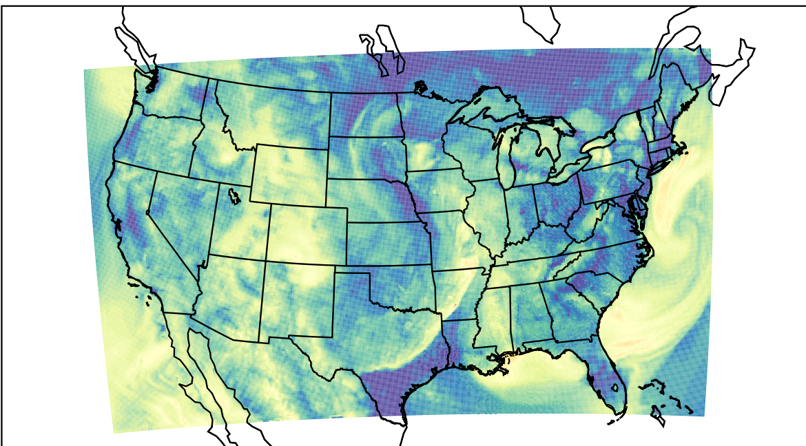
WRF (2019-10-21_11:00:00)
