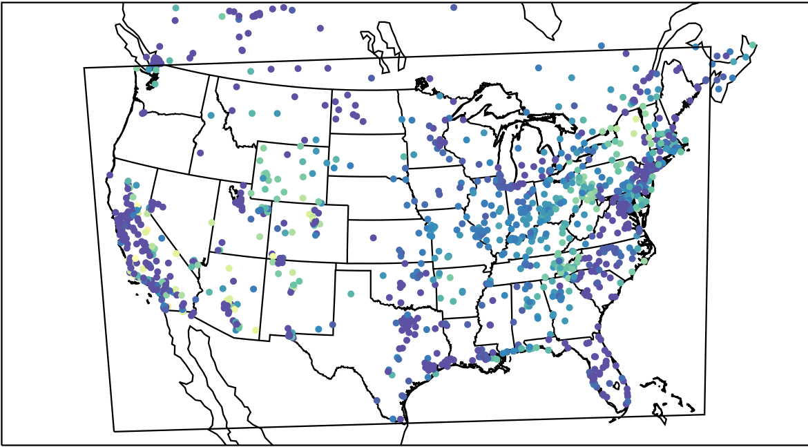
AirNOW (2019-10-22_14:00:00)
