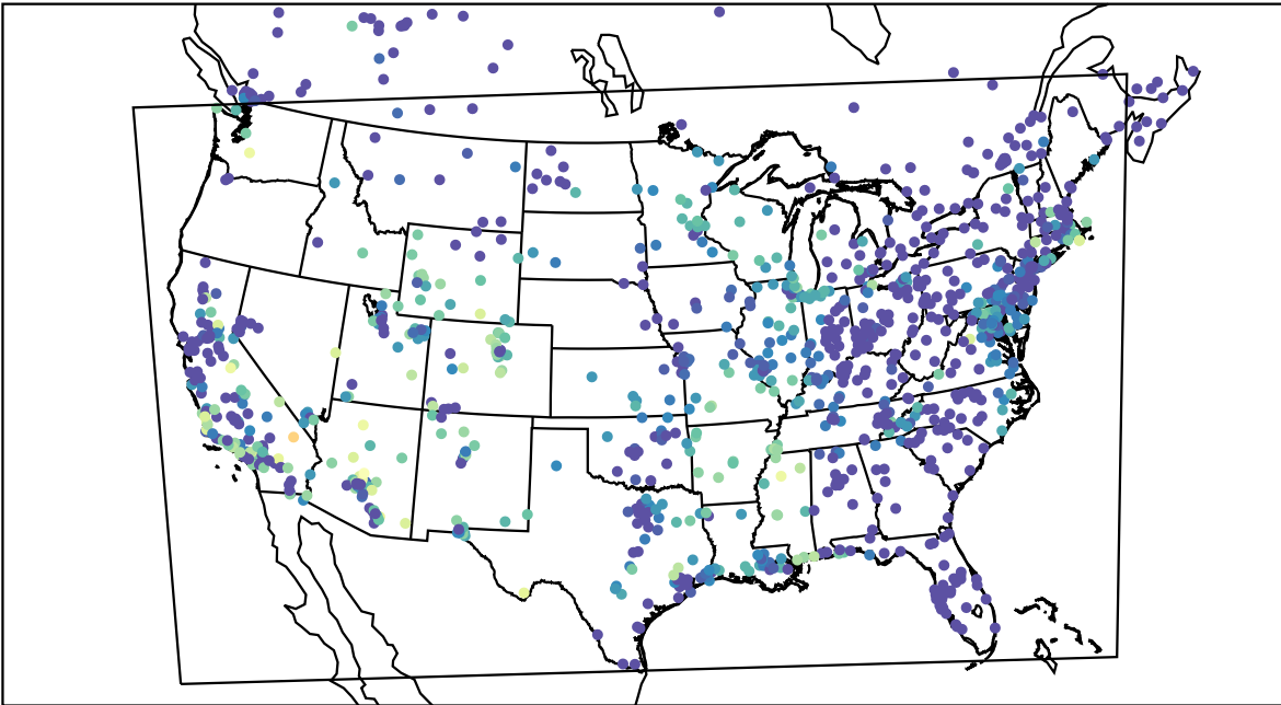
AirNOW (2019-10-21_11:00:00)
