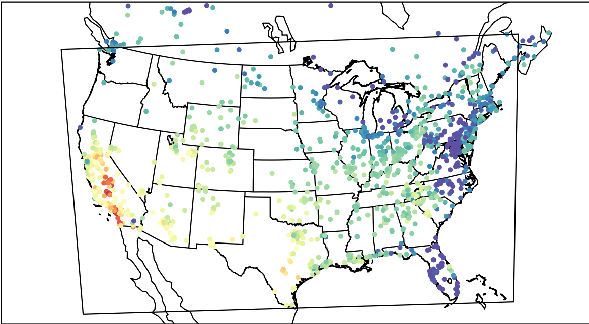
AirNOW (2019-10-22_22:00:00)
