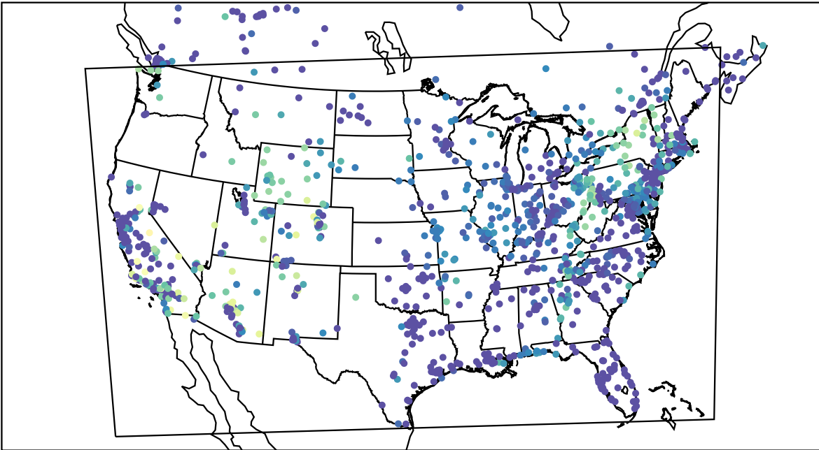
AirNOW (2019-10-22_12:00:00)
