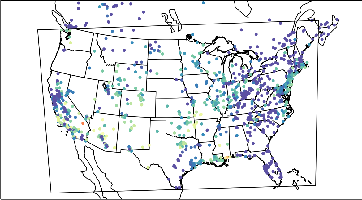
AirNOW (2019-10-21_06:00:00)
