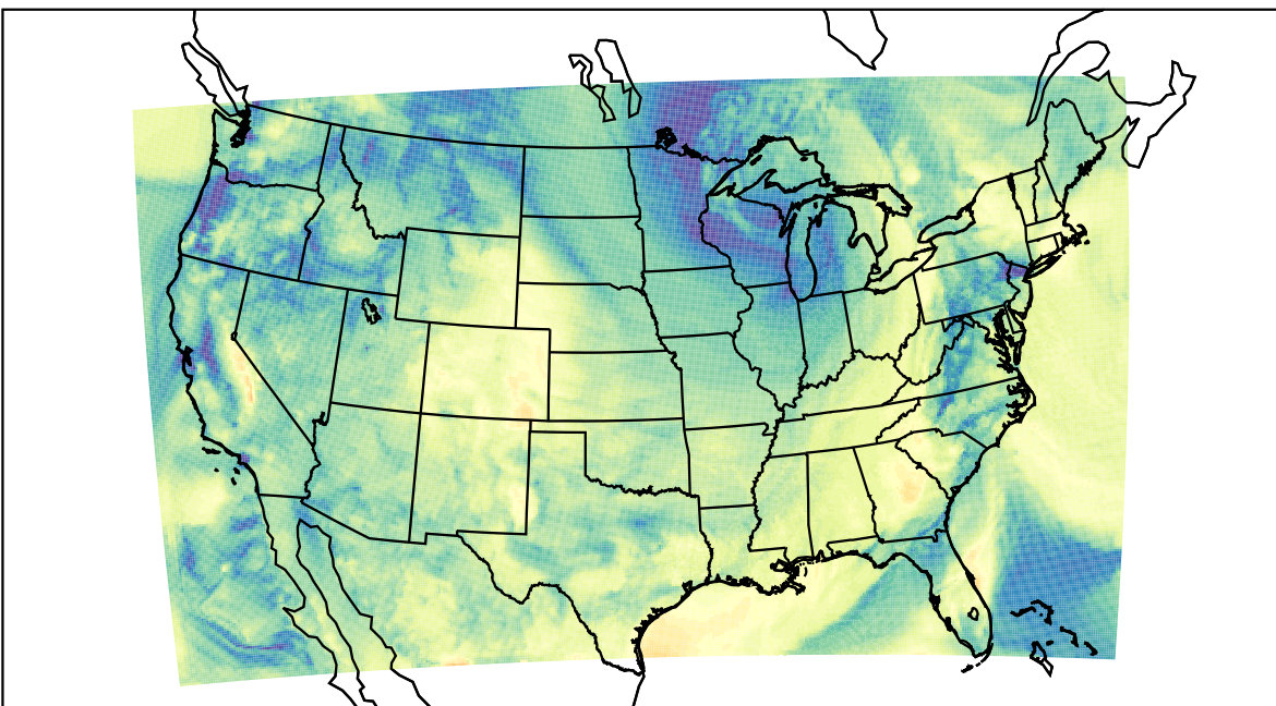
WRF (2019-10-22_17:00:00)
