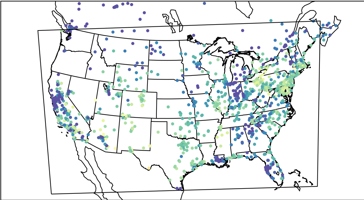
AirNOW (2019-10-21_16:00:00)
