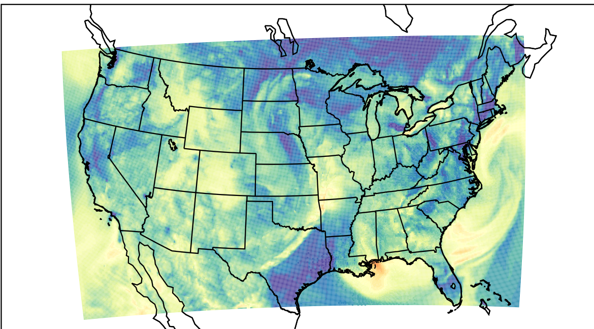
WRF (2019-10-21_07:00:00)
