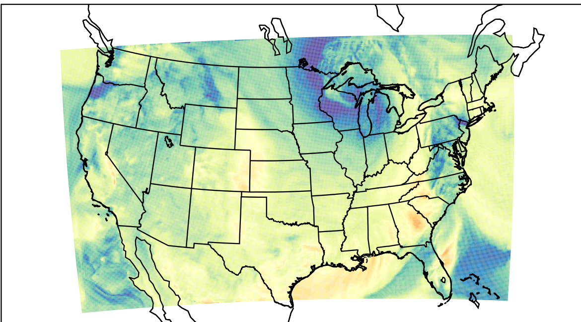
WRF (2019-10-22_19:00:00)
