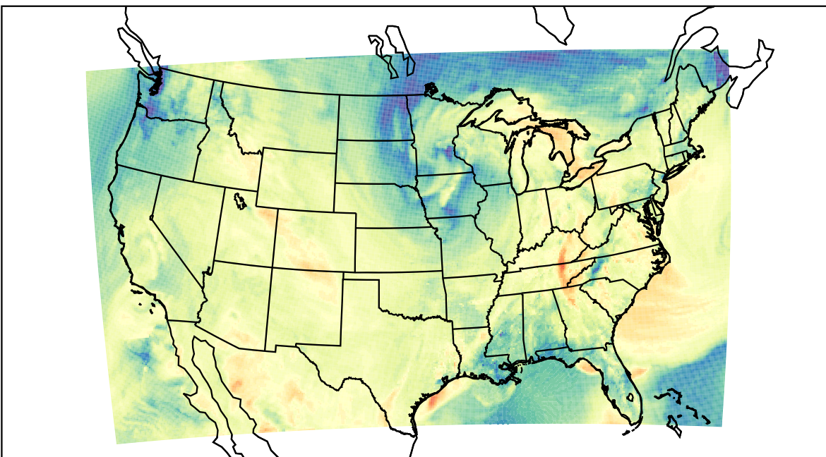
WRF (2019-10-21_22:00:00)
