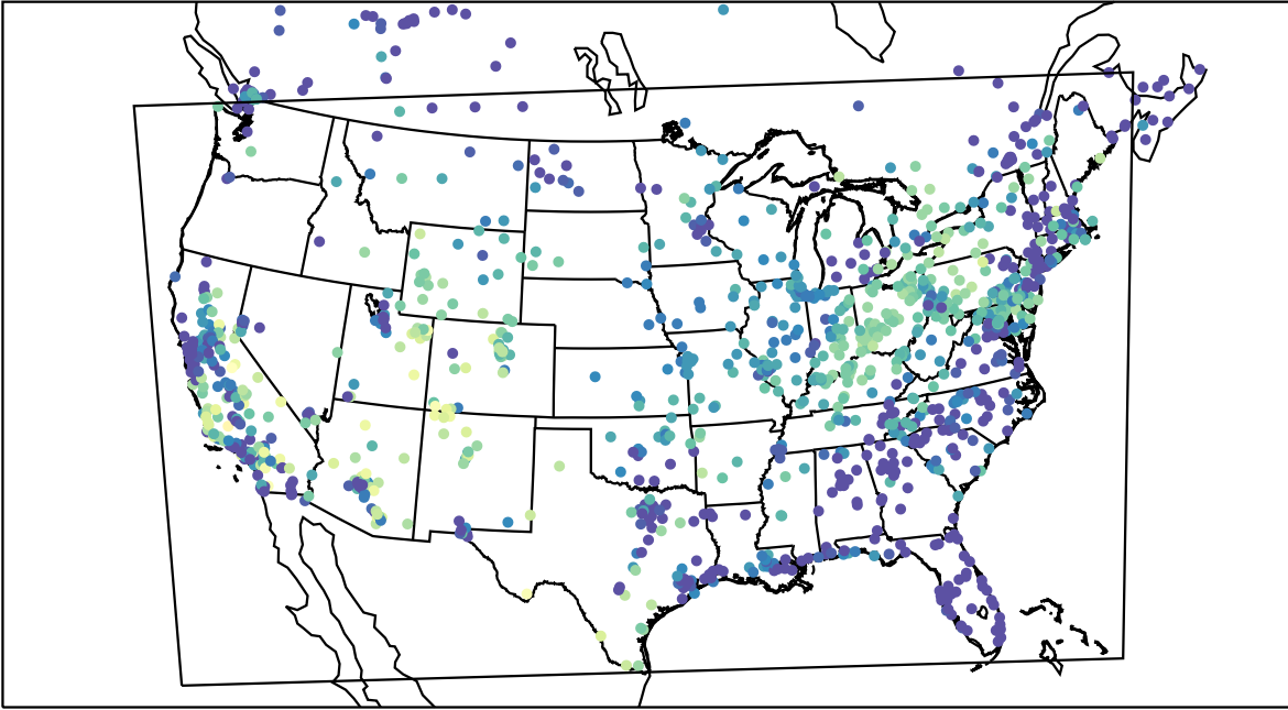
AirNOW (2019-10-22_03:00:00)
