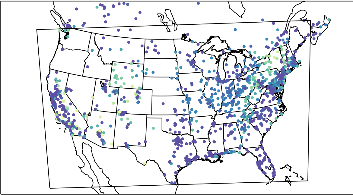
AirNOW (2019-10-22_13:00:00)
