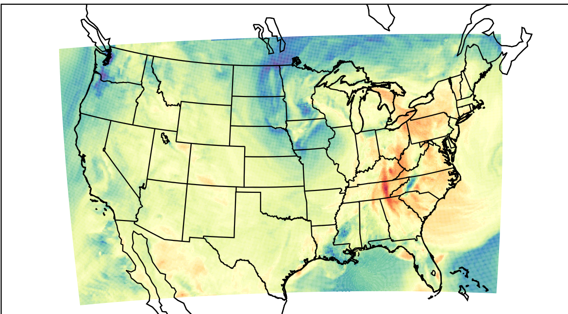
WRF (2019-10-21_20:00:00)
