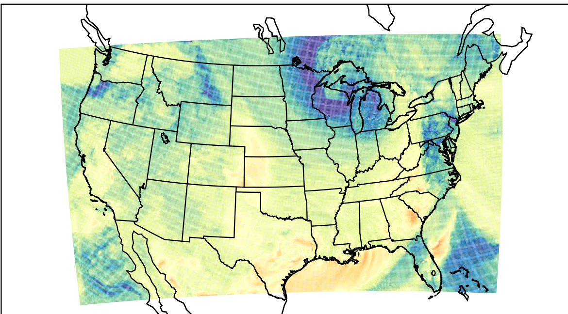
WRF (2019-10-22_21:00:00)
