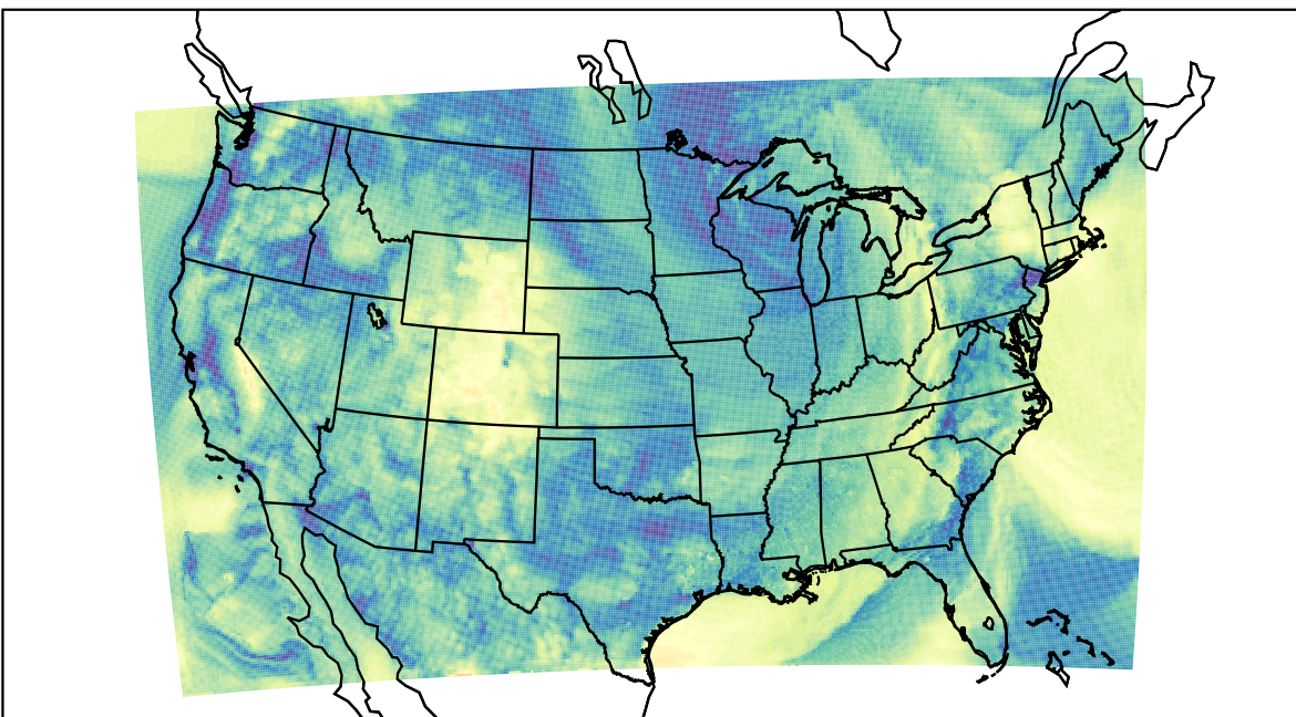
WRF (2019-10-22_15:00:00)
