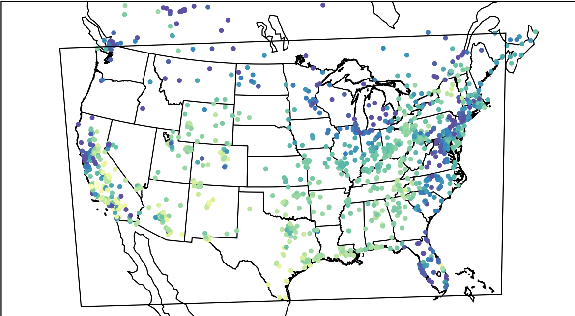
AirNOW (2019-10-22_17:00:00)
