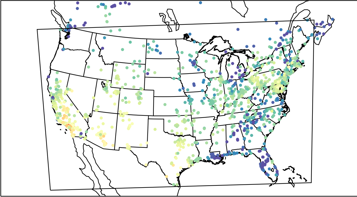
AirNOW (2019-10-21_21:00:00)
