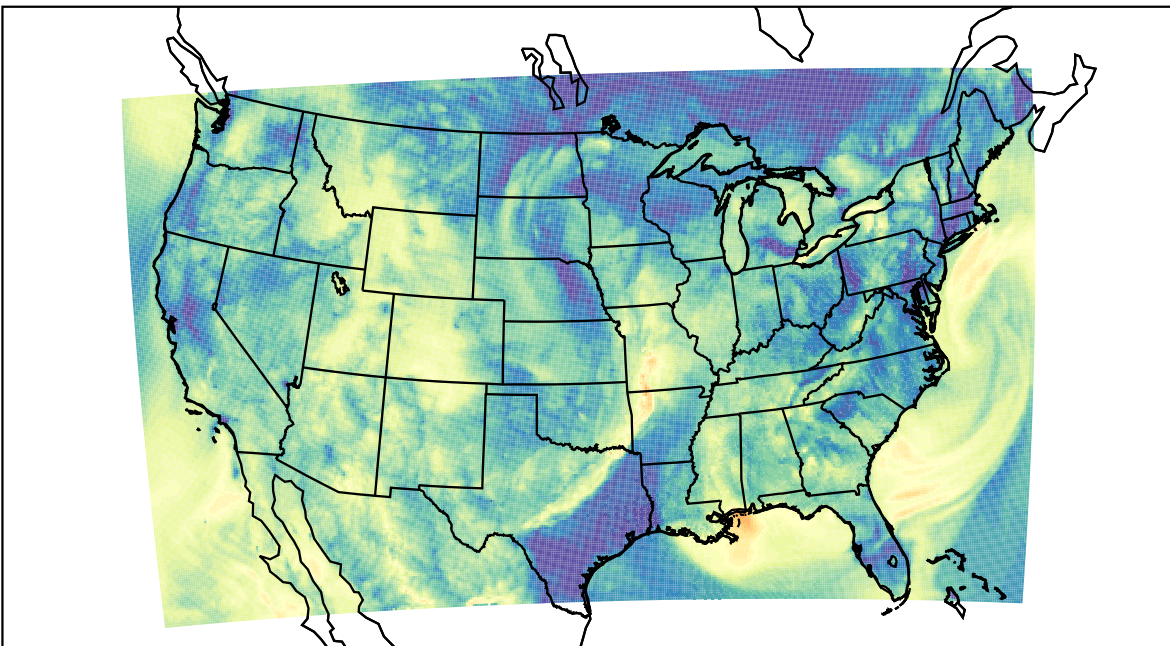
WRF (2019-10-21_08:00:00)
