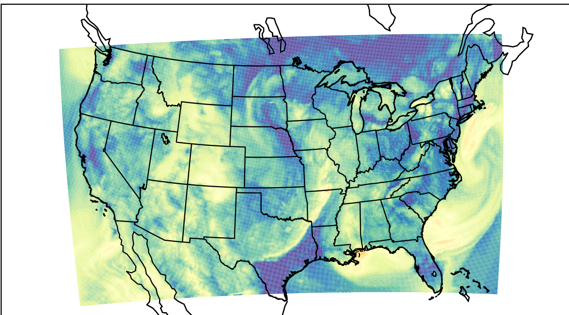
WRF (2019-10-21_10:00:00)
