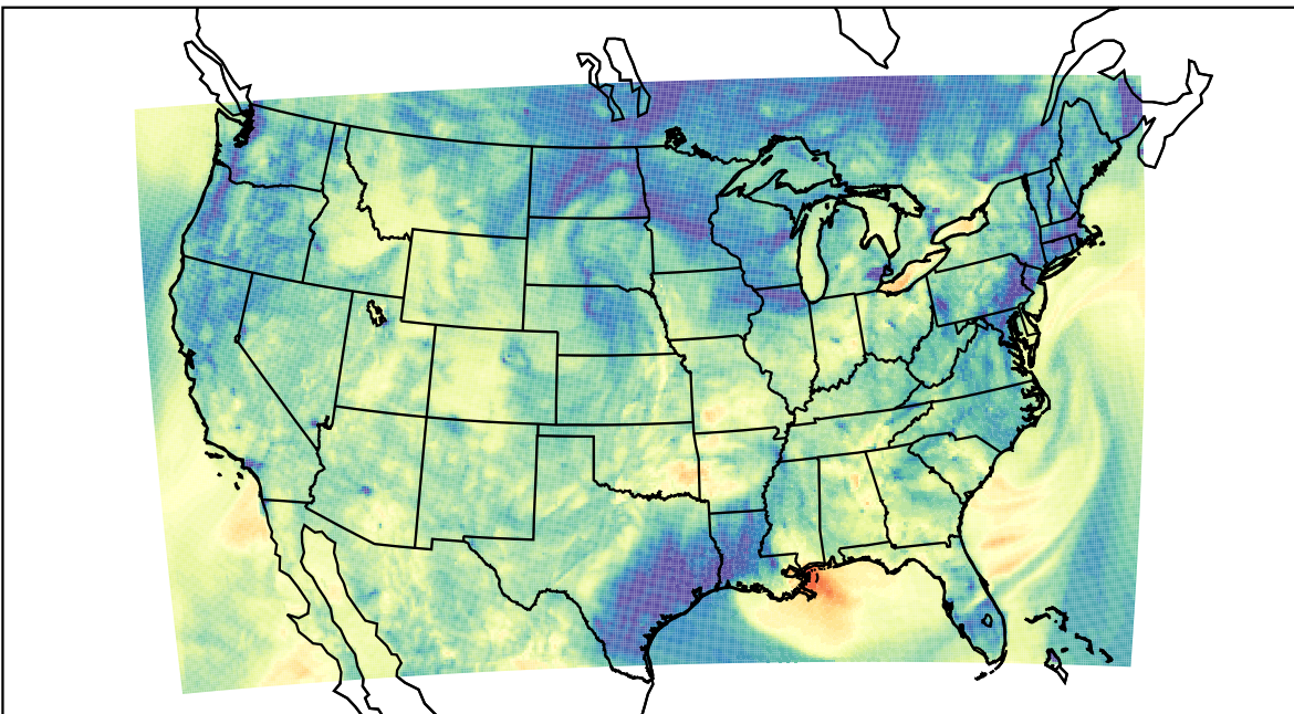
WRF (2019-10-21_03:00:00)
