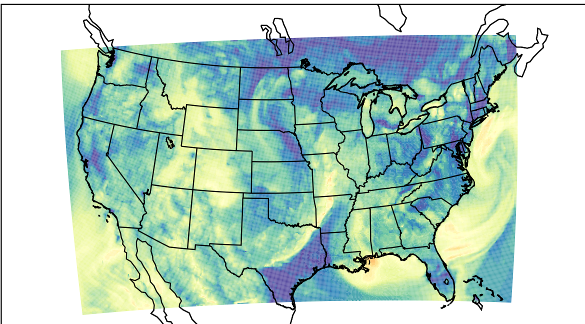
WRF (2019-10-21_09:00:00)
