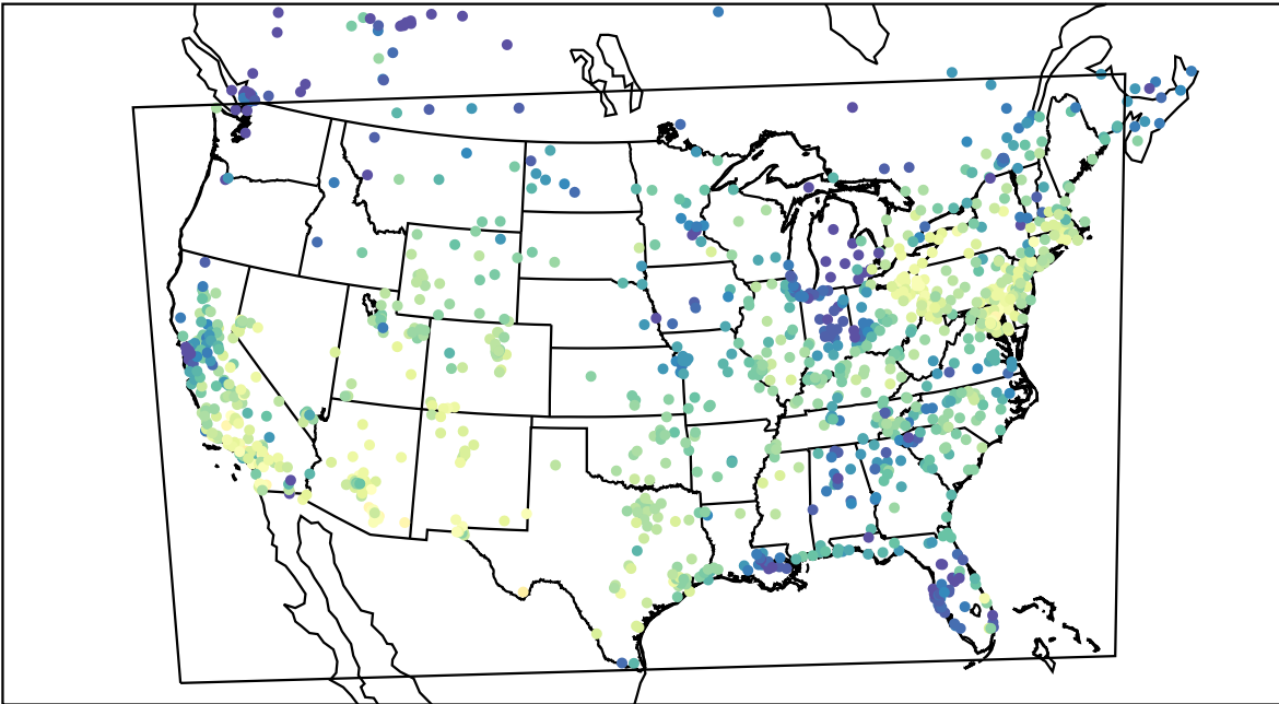
AirNOW (2019-10-21_18:00:00)
