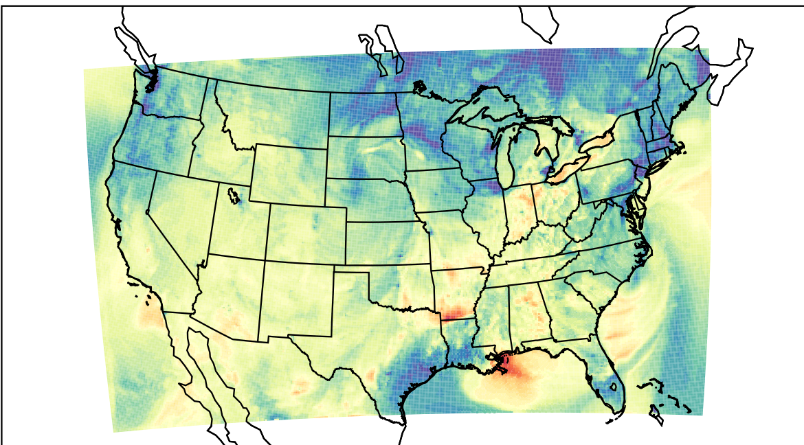
WRF (2019-10-21_00:00:00)
