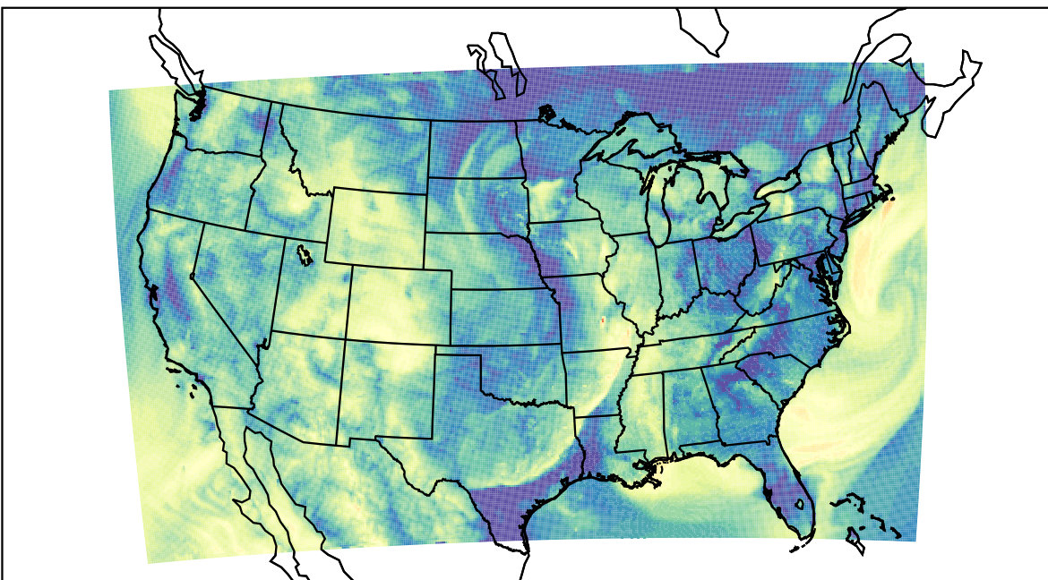
WRF (2019-10-21_12:00:00)
