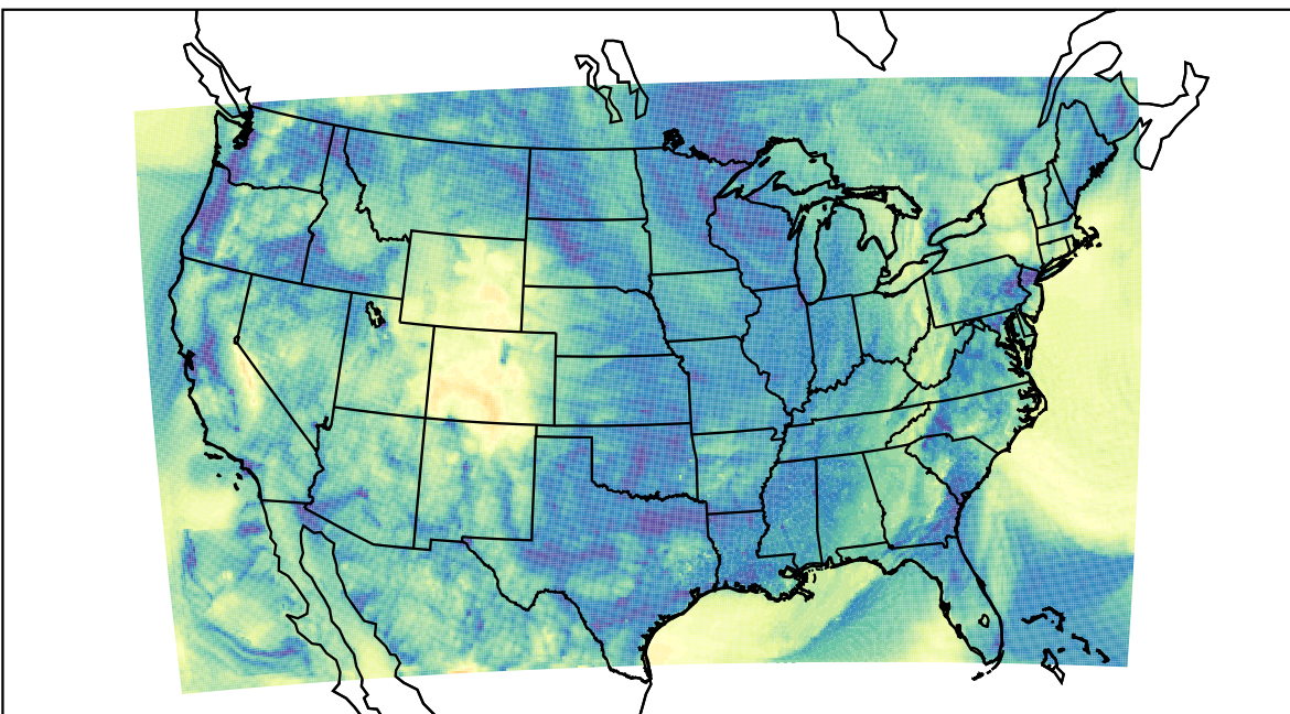
WRF (2019-10-22_14:00:00)
