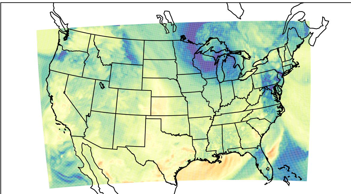
WRF (2019-10-22_22:00:00)
