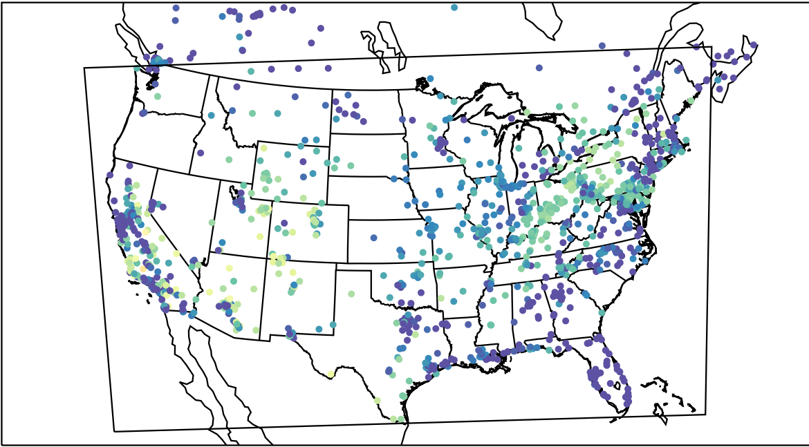
AirNOW (2019-10-22_04:00:00)
