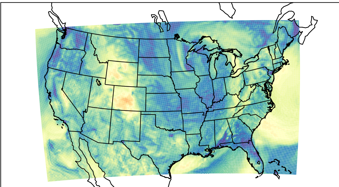
WRF (2019-10-22_08:00:00)
