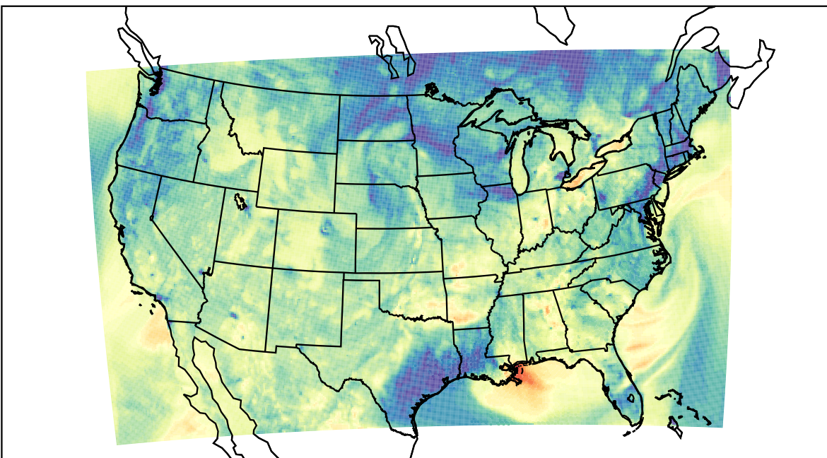
WRF (2019-10-21_02:00:00)
