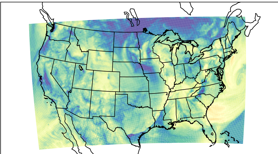
WRF (2019-10-21_15:00:00)
