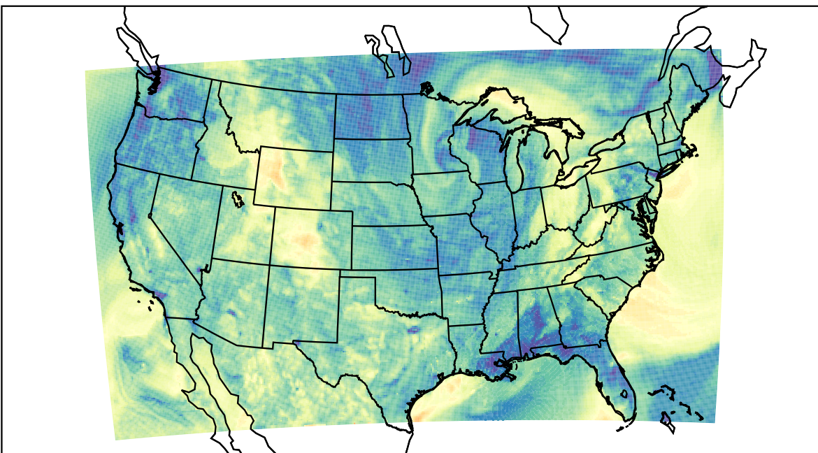
WRF (2019-10-22_04:00:00)
