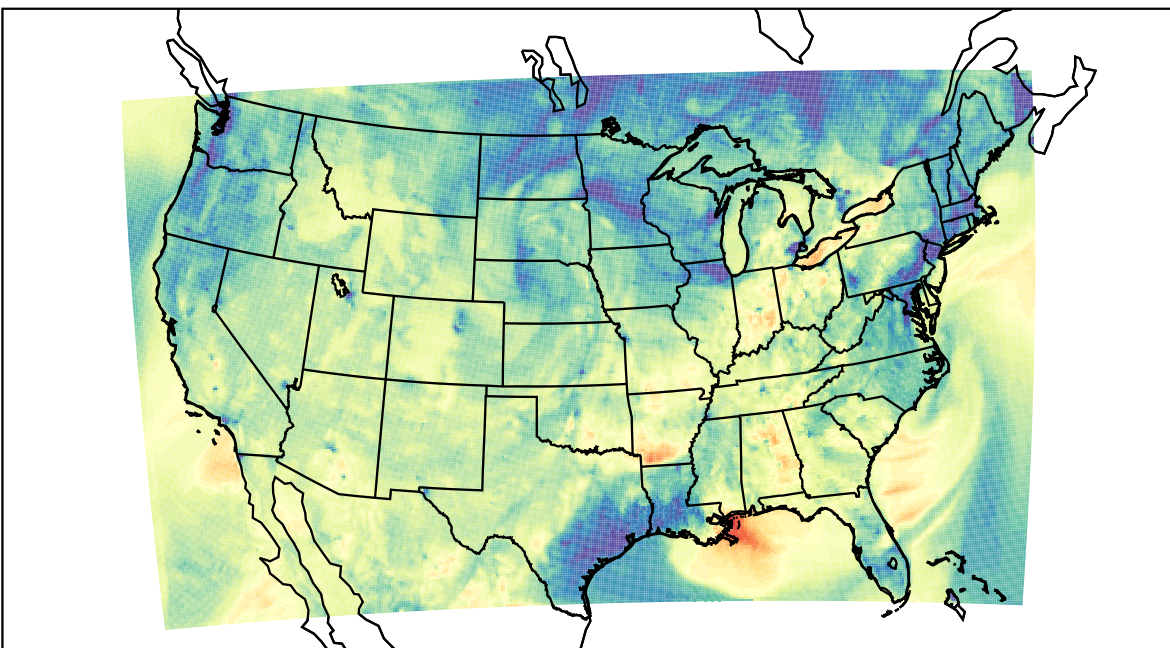
WRF (2019-10-21_01:00:00)
