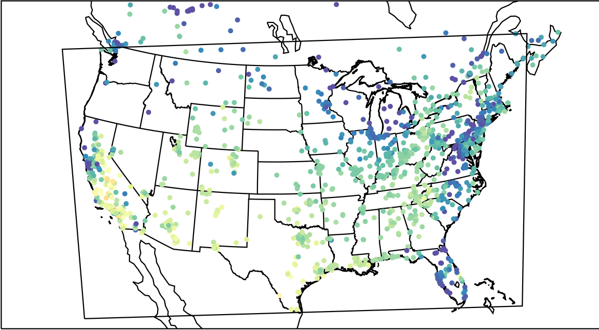
AirNOW (2019-10-22_18:00:00)
