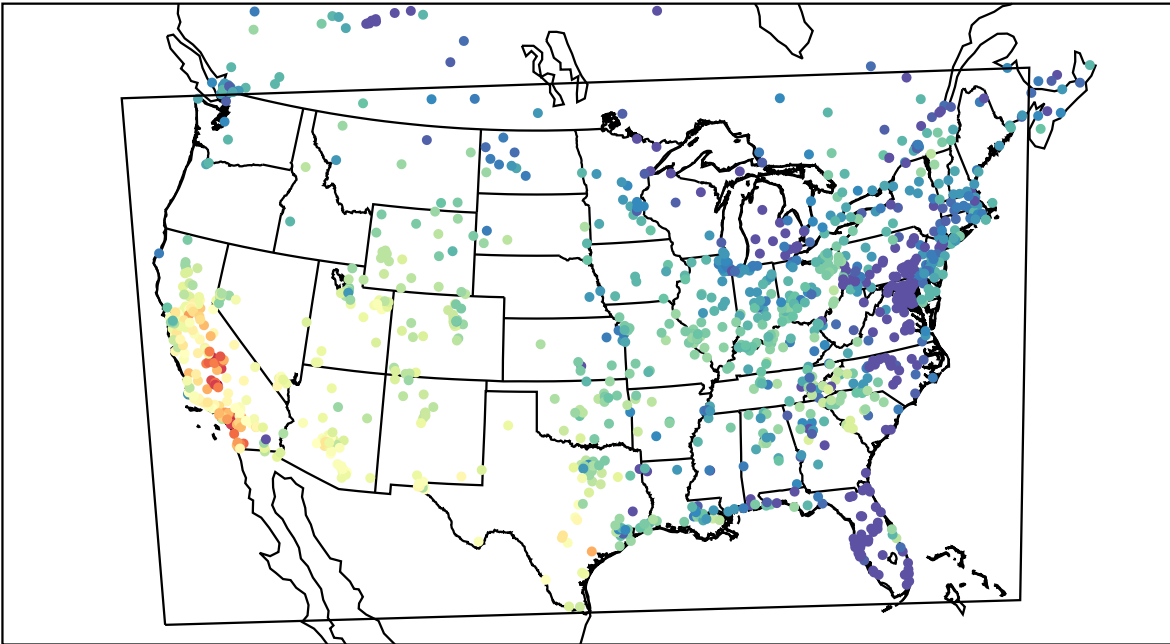
AirNOW (2019-10-22_23:00:00)
