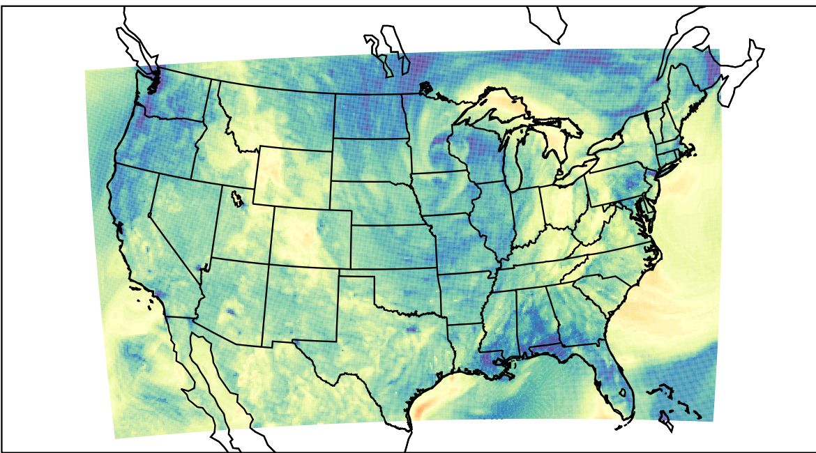
WRF (2019-10-22_02:00:00)
