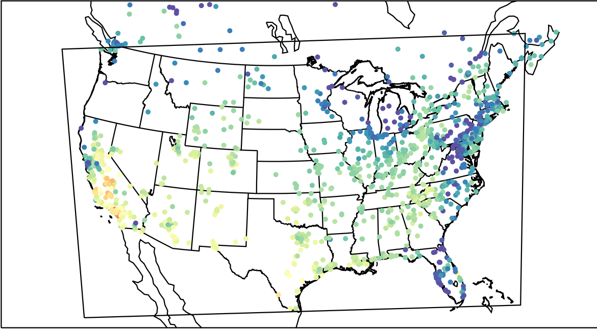
AirNOW (2019-10-22_19:00:00)
