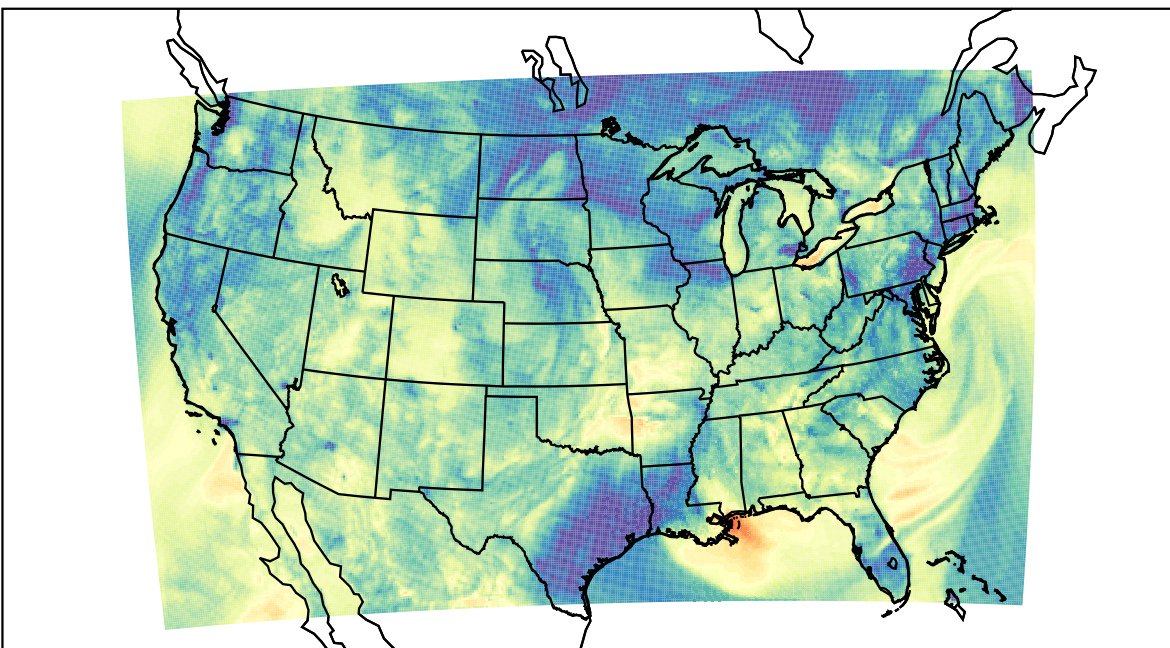
WRF (2019-10-21_04:00:00)
