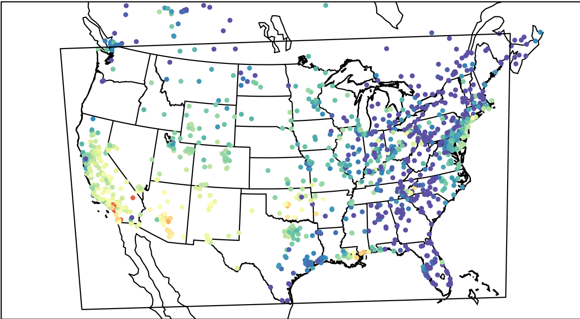
AirNOW (2019-10-21_00:00:00)
