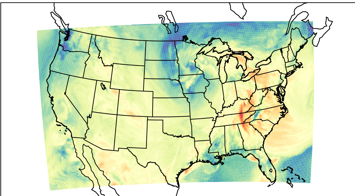
WRF (2019-10-21_21:00:00)
