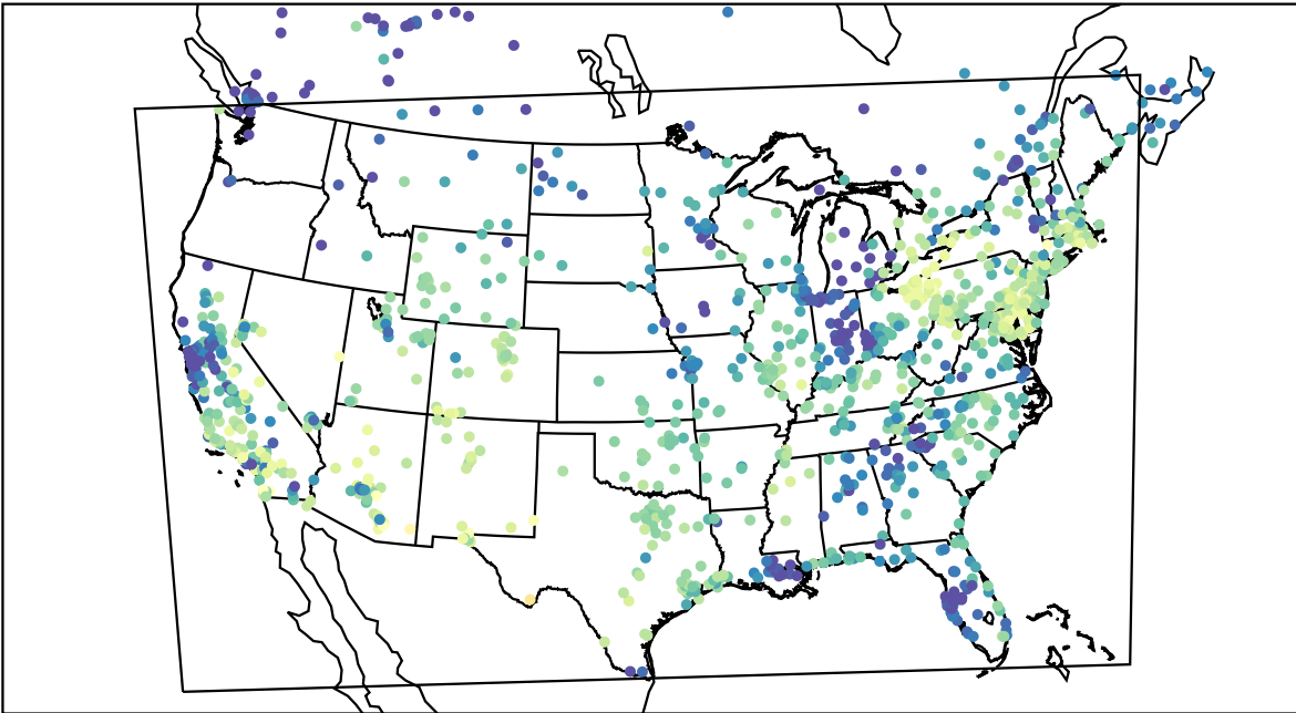
AirNOW (2019-10-21_17:00:00)
