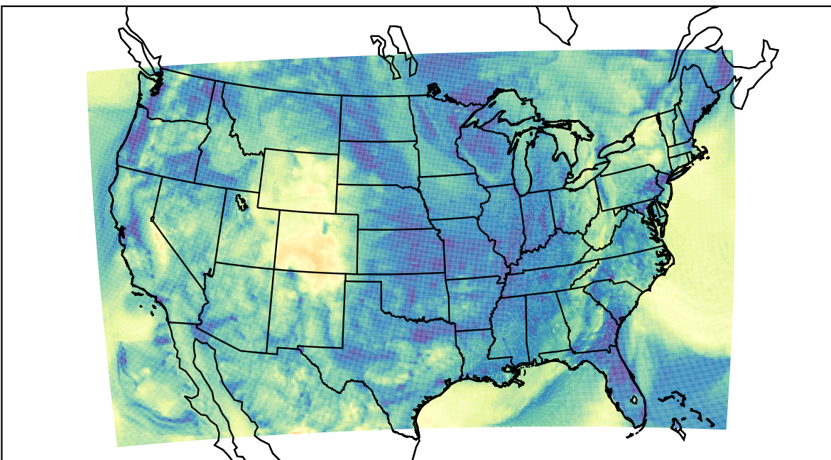
WRF (2019-10-22_13:00:00)
