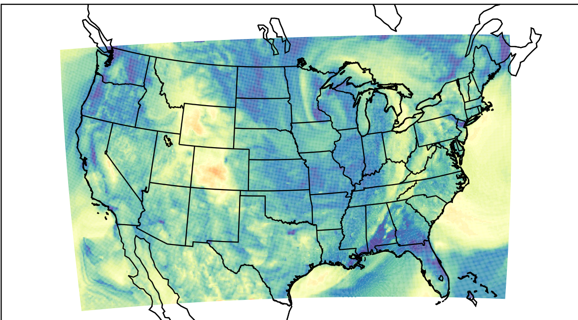
WRF (2019-10-22_07:00:00)
