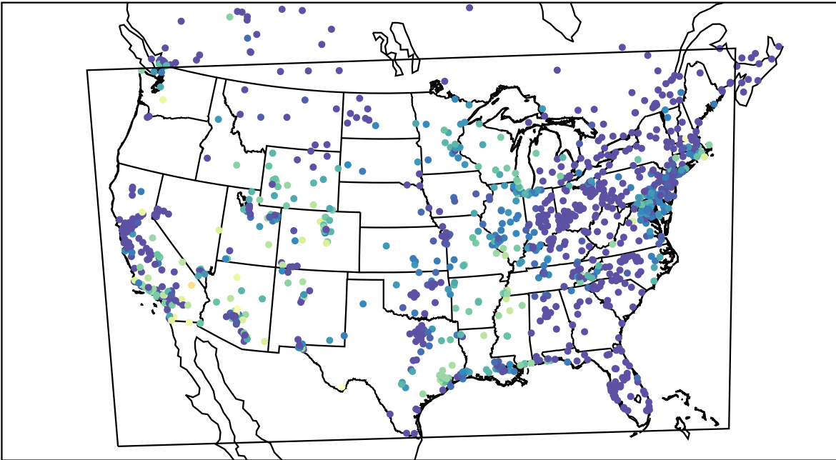
AirNOW (2019-10-21_12:00:00)
