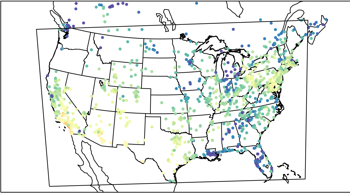
AirNOW (2019-10-21_20:00:00)
