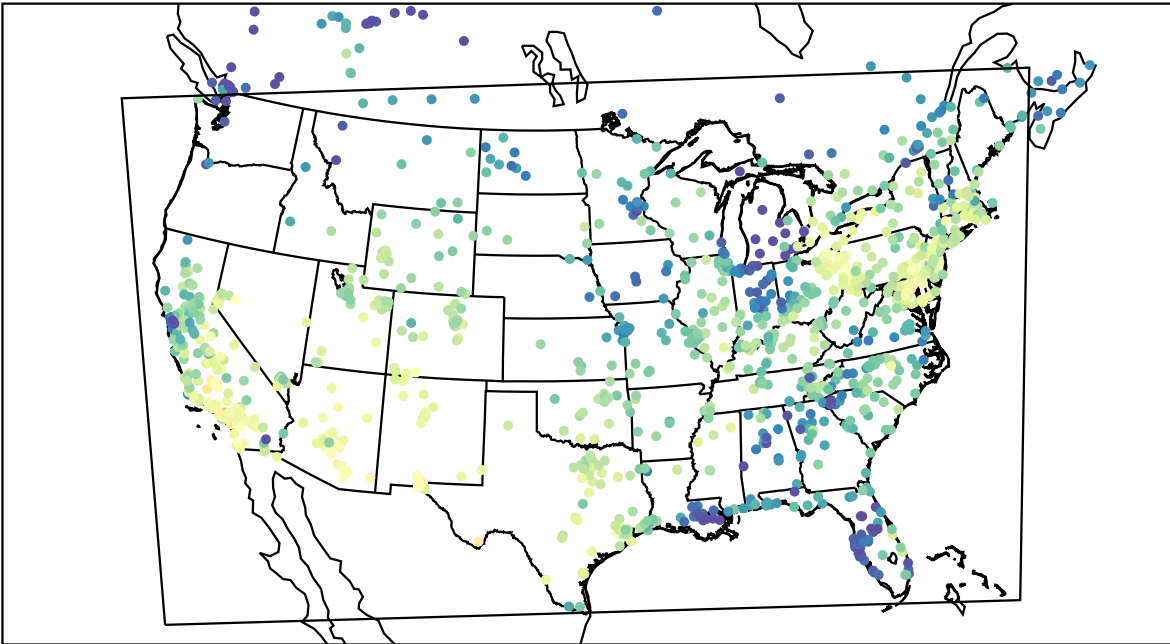
AirNOW (2019-10-21_19:00:00)
