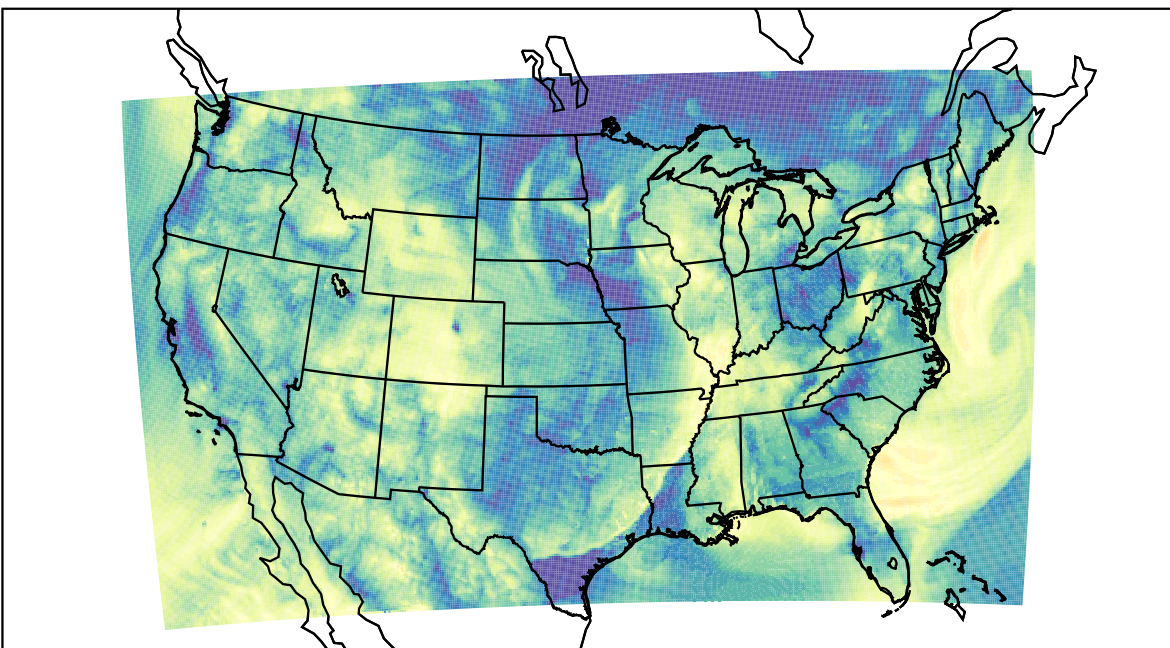
WRF (2019-10-21_14:00:00)
