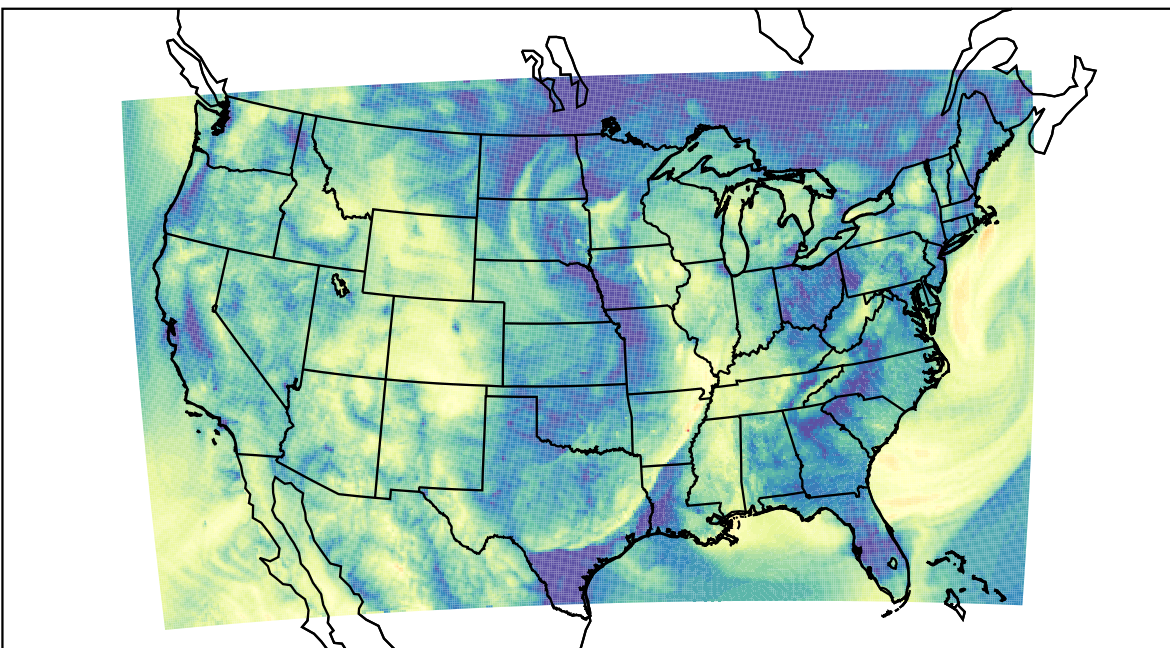
WRF (2019-10-21_13:00:00)
