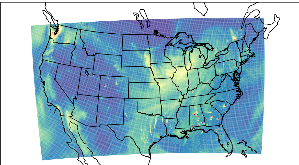
WRF 2019-11-04_21:00:00
