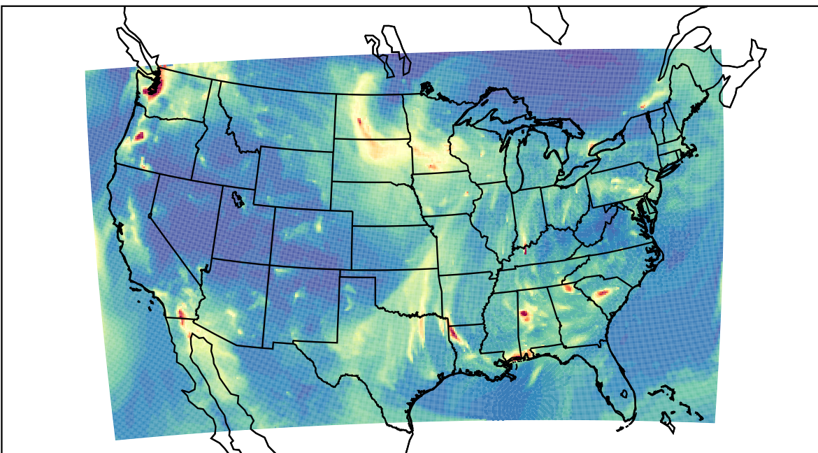
WRF 2019-11-04_06:00:00
