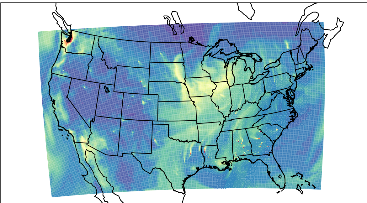
WRF 2019-11-04_18:00:00
