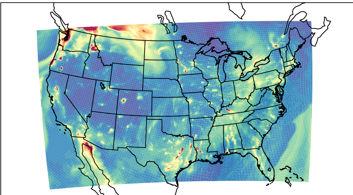
WRF 2019-11-03_03:00:00
