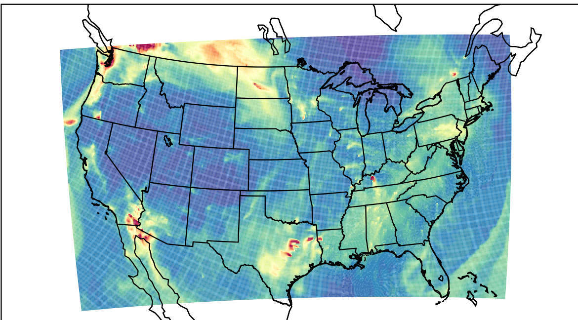
WRF 2019-11-03_10:00:00
