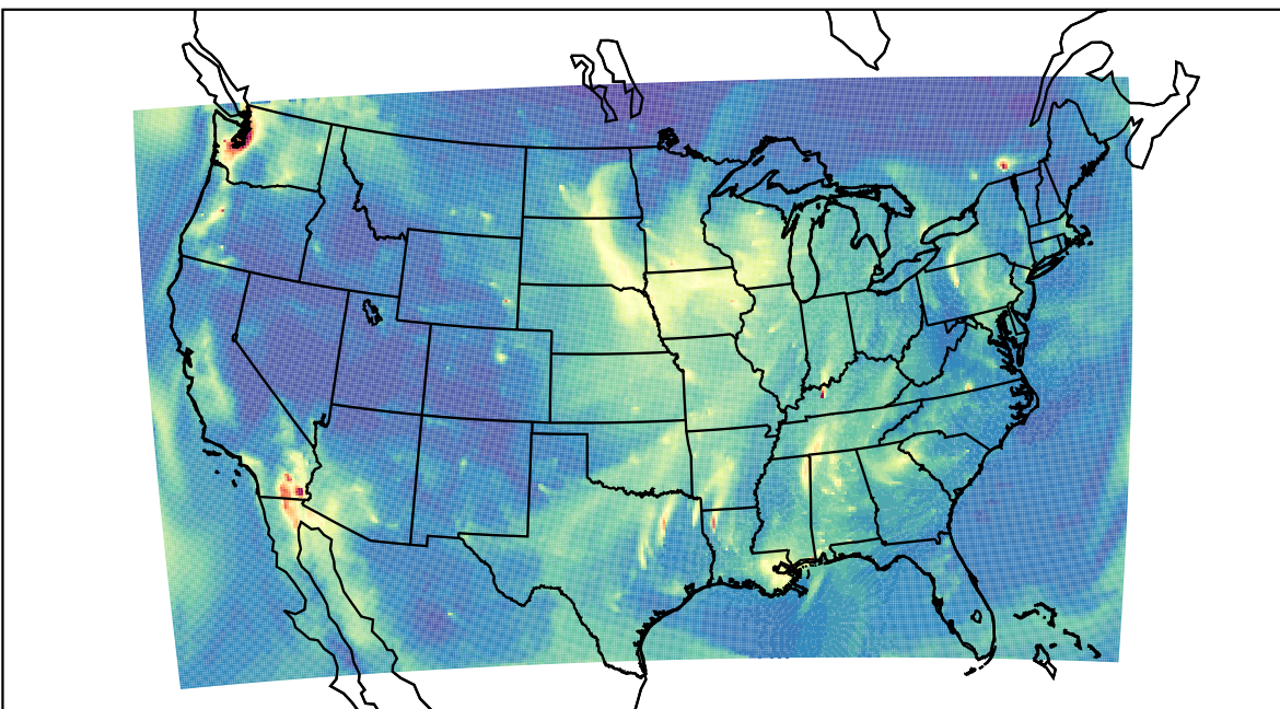
WRF 2019-11-04_14:00:00
