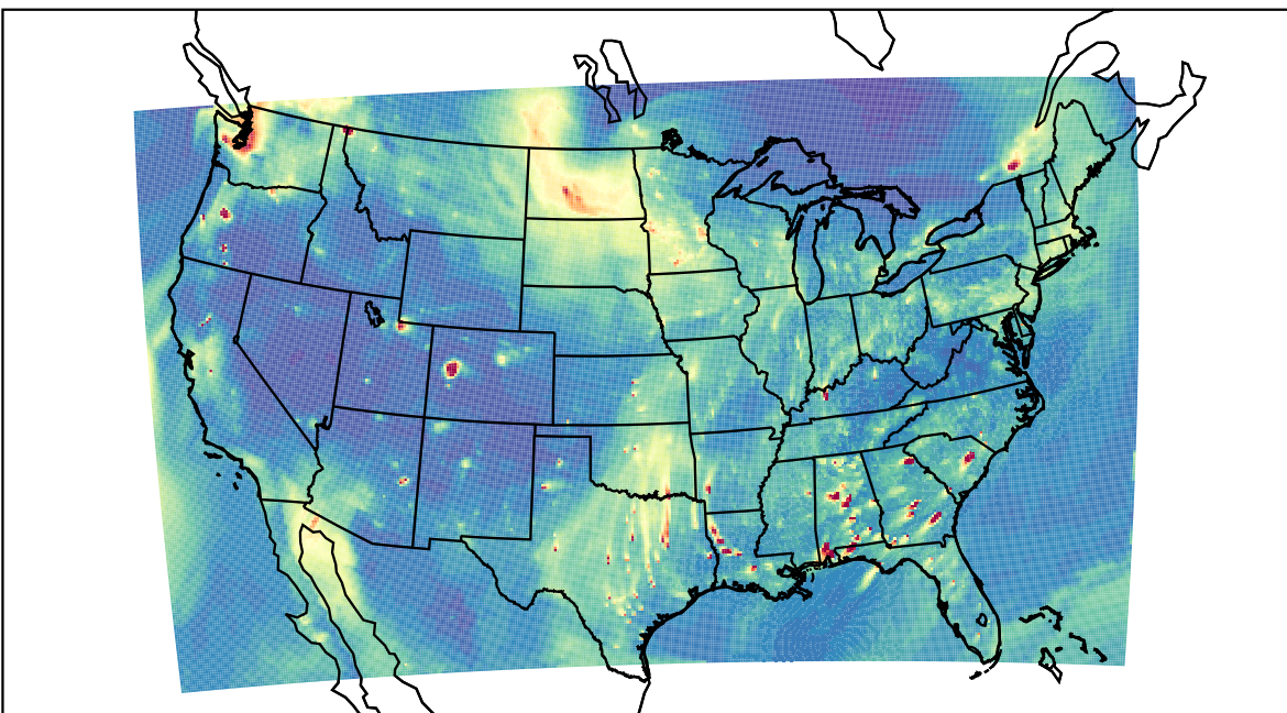
WRF 2019-11-04_00:00:00
