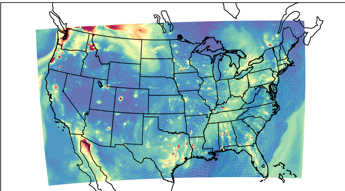
WRF 2019-11-03_02:00:00
