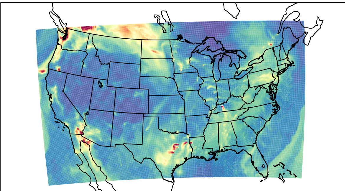
WRF 2019-11-03_09:00:00
