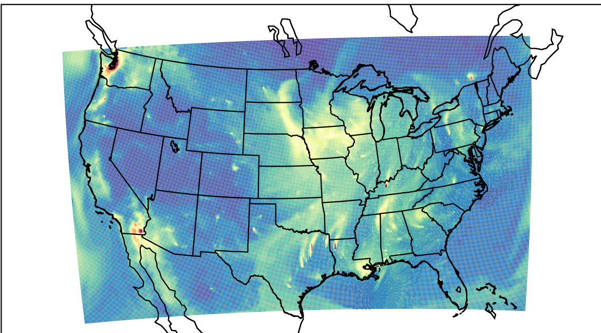
WRF 2019-11-04_15:00:00
