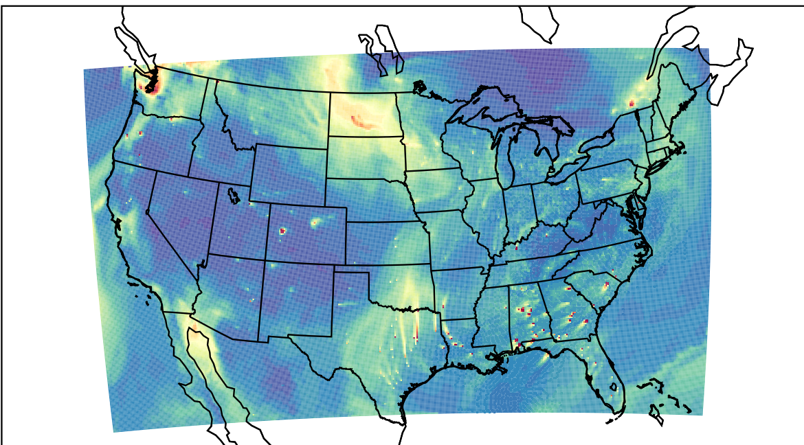
WRF 2019-11-03_22:00:00
