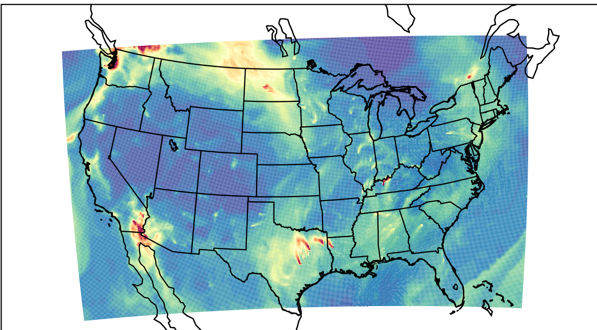
WRF 2019-11-03_15:00:00
