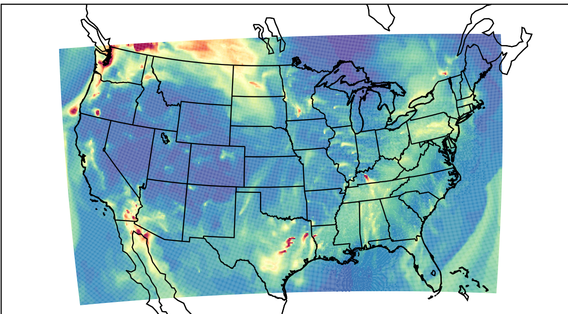
WRF 2019-11-03_07:00:00
