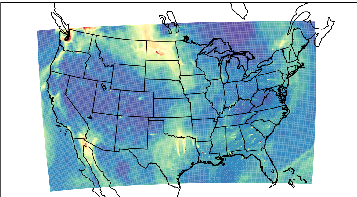
WRF 2019-11-03_19:00:00
