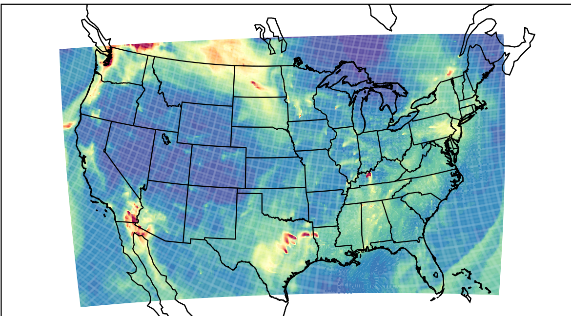
WRF 2019-11-03_12:00:00
