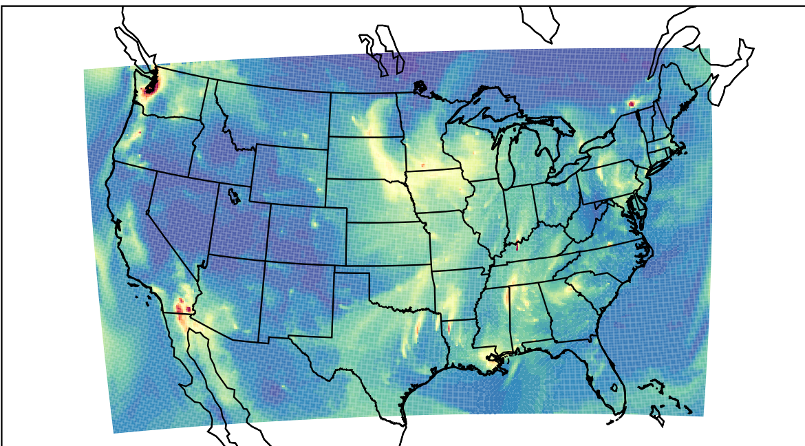
WRF 2019-11-04_13:00:00
