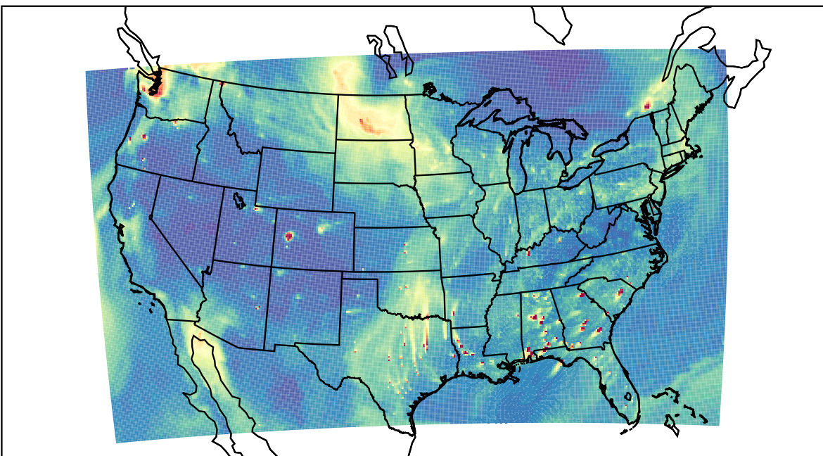
WRF 2019-11-03_23:00:00
