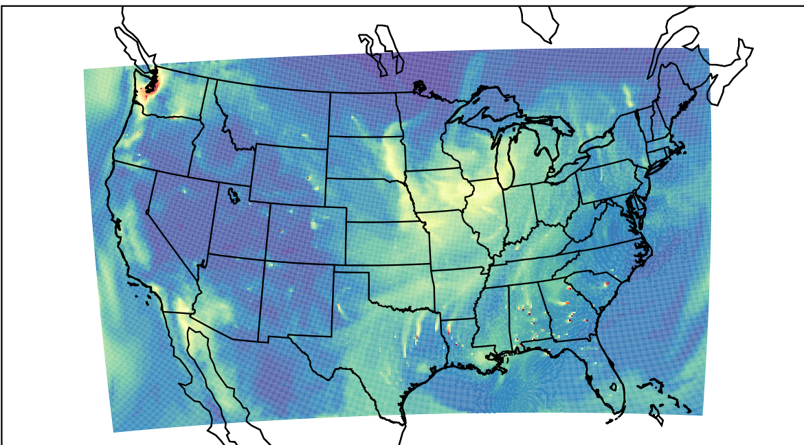
WRF 2019-11-04_19:00:00
