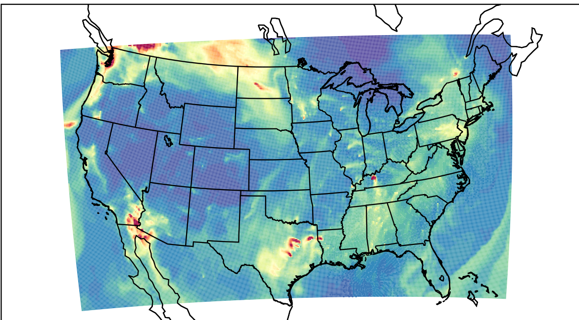
WRF 2019-11-03_11:00:00
