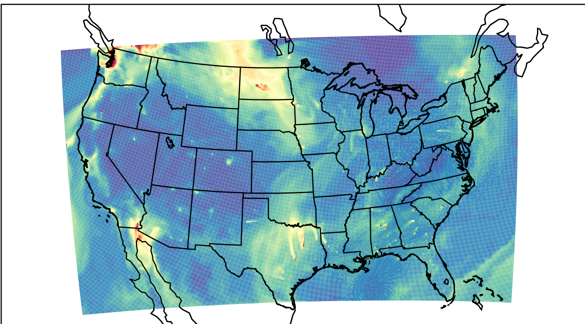
WRF 2019-11-03_18:00:00
