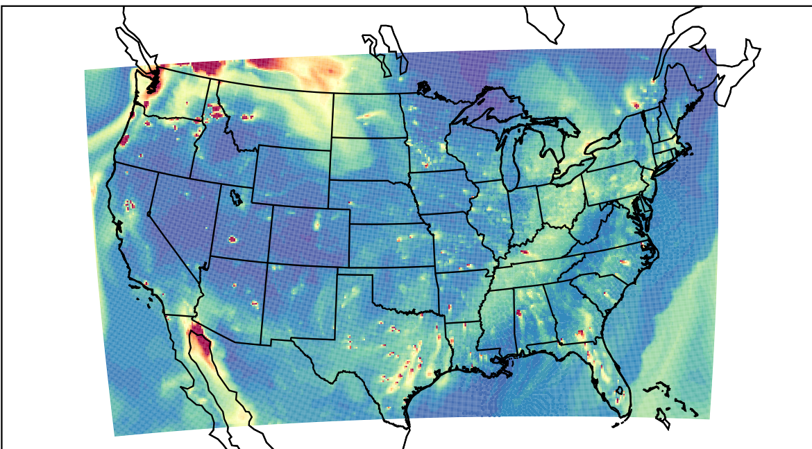
WRF 2019-11-03_00:00:00
