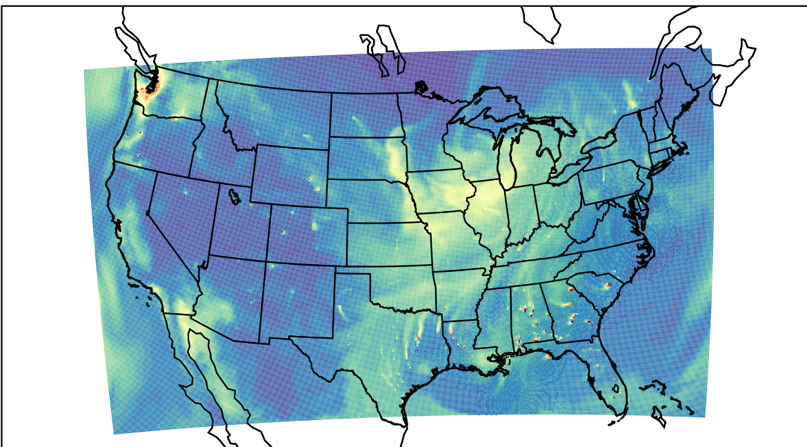
WRF 2019-11-04_20:00:00
