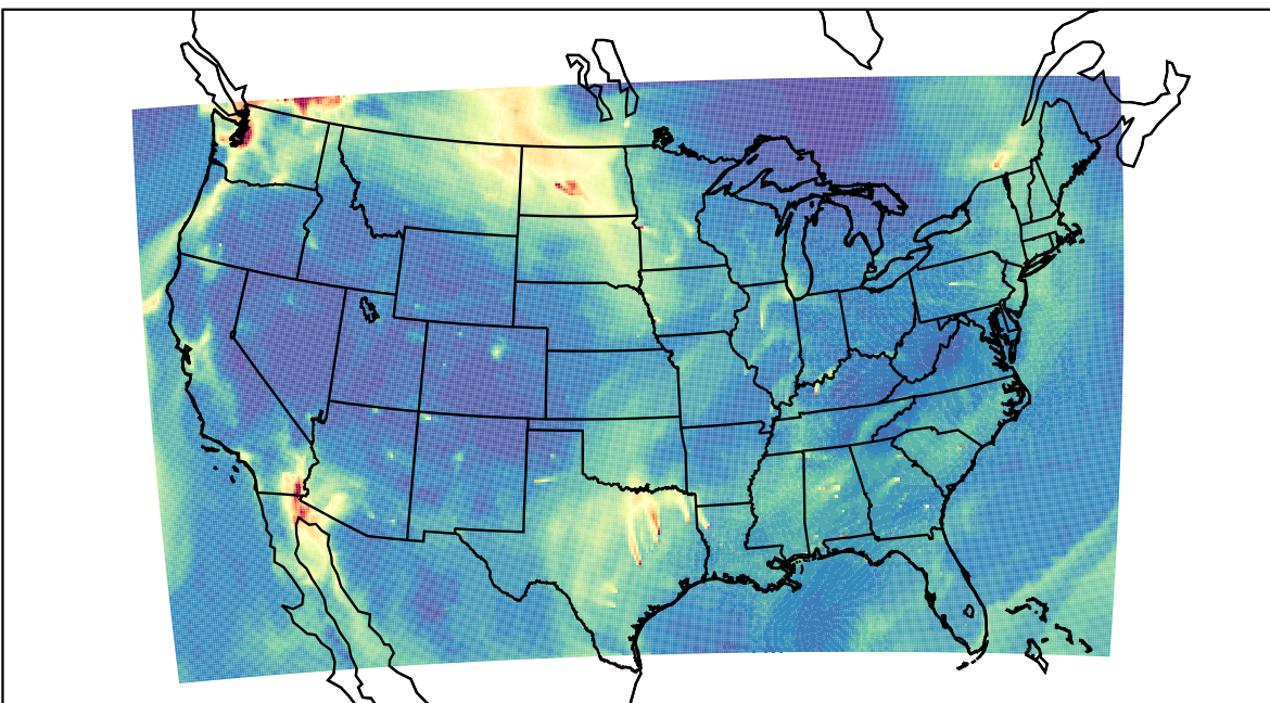
WRF 2019-11-03_17:00:00
