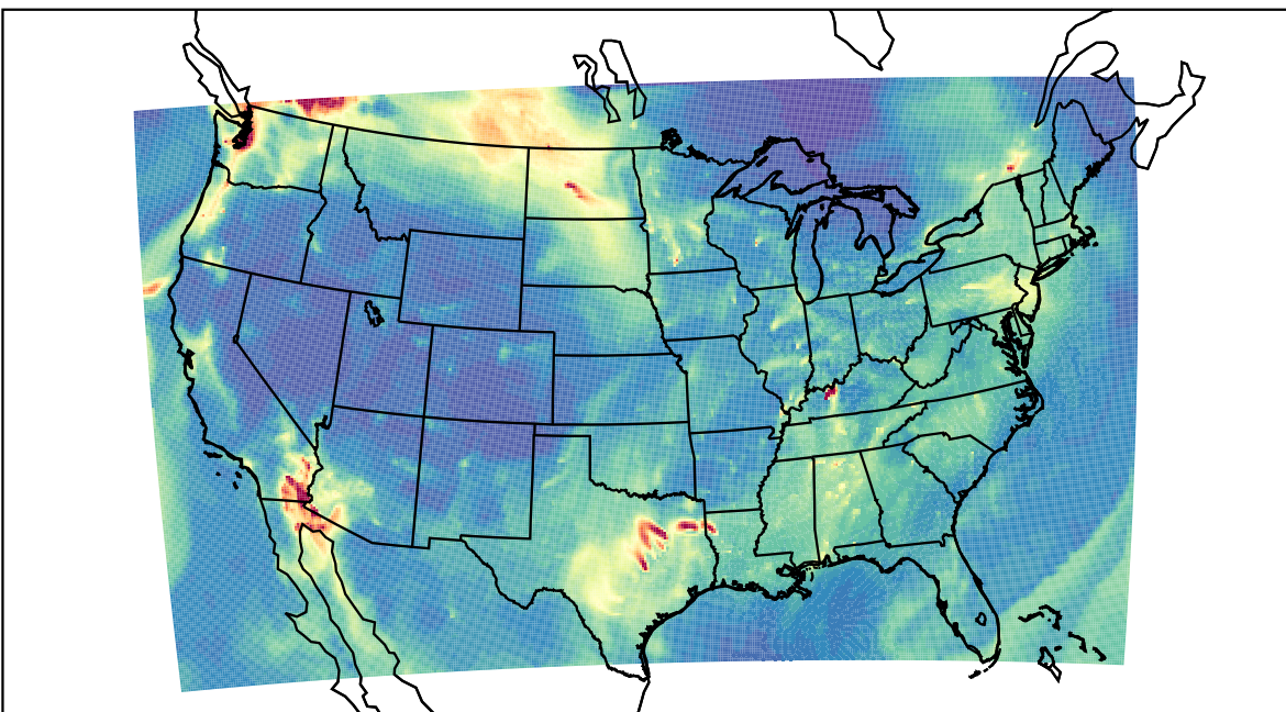
WRF 2019-11-03_13:00:00
