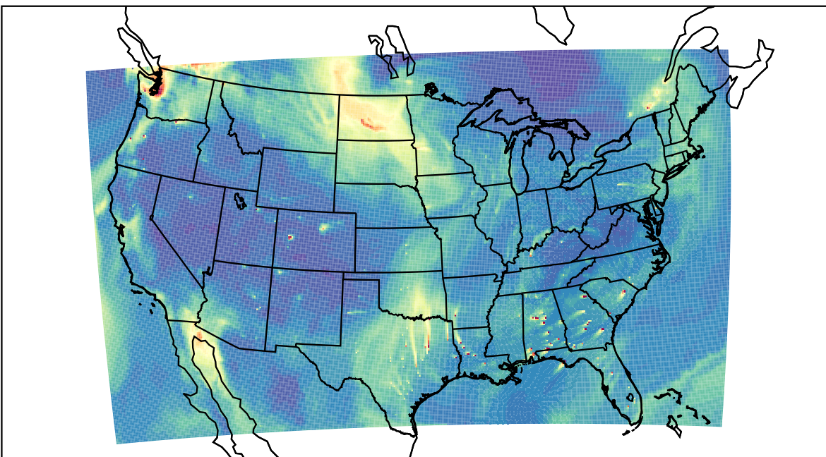
WRF 2019-11-03_21:00:00
