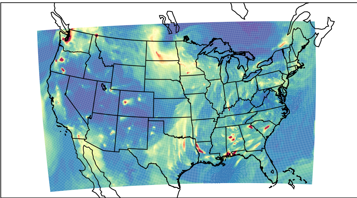
WRF 2019-11-04_03:00:00
