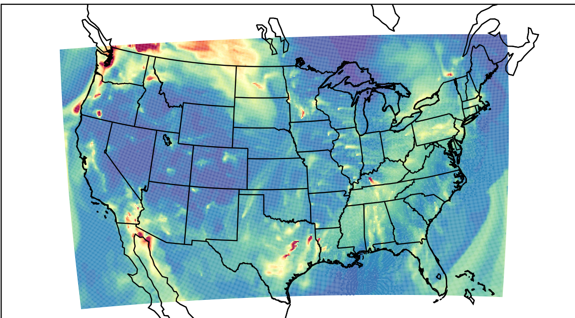
WRF 2019-11-03_06:00:00
