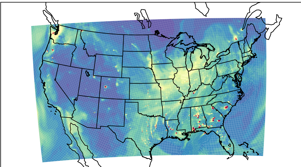
WRF 2019-11-04_23:00:00
