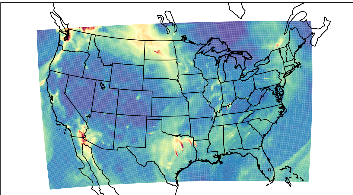
WRF 2019-11-03_16:00:00
