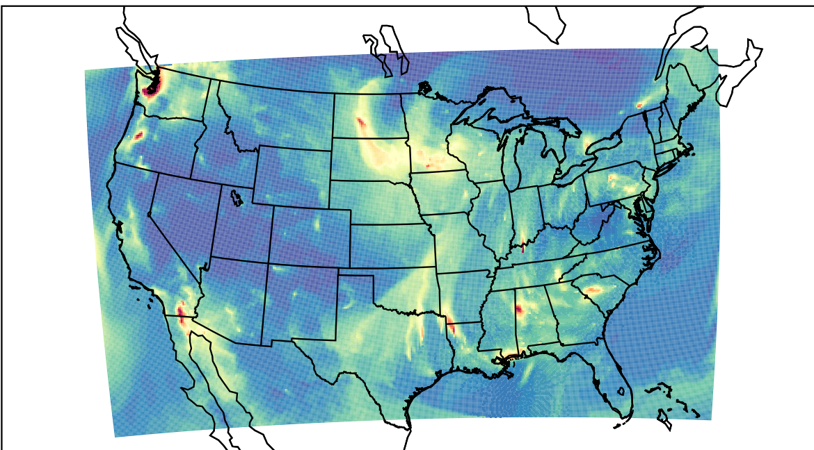
WRF 2019-11-04_08:00:00
