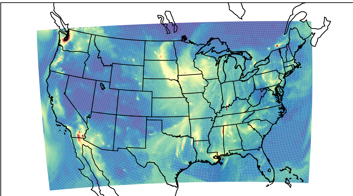
WRF 2019-11-04_12:00:00
