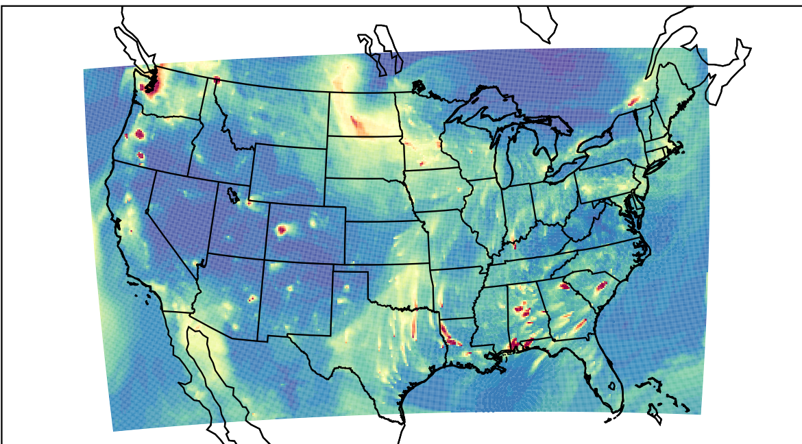
WRF 2019-11-04_02:00:00
