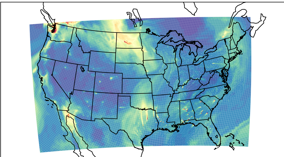
WRF 2019-11-03_20:00:00
