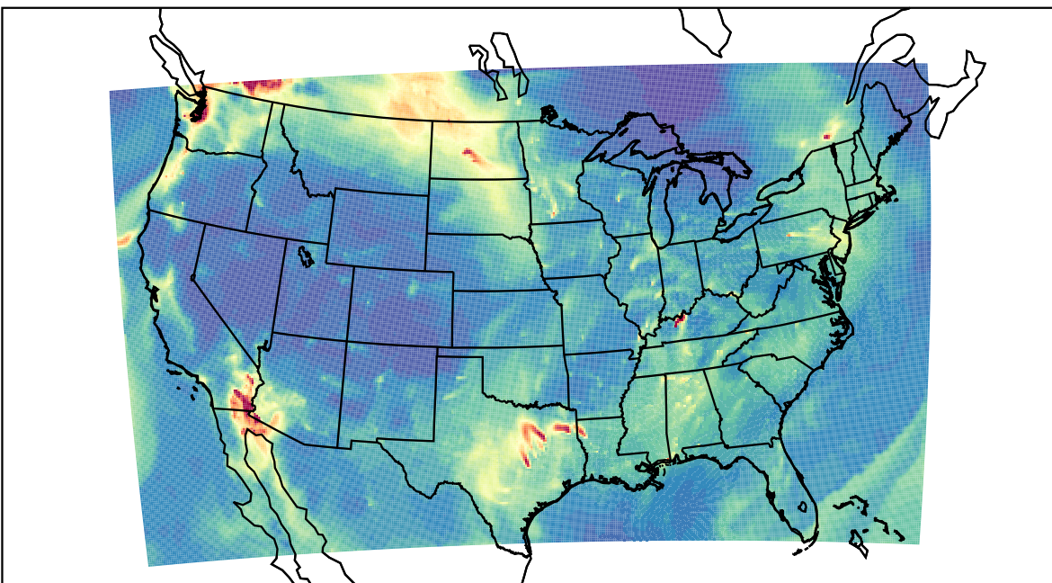
WRF 2019-11-03_14:00:00
