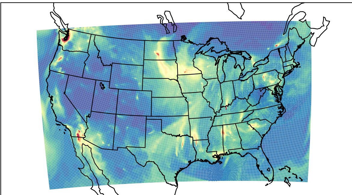
WRF 2019-11-04_10:00:00
