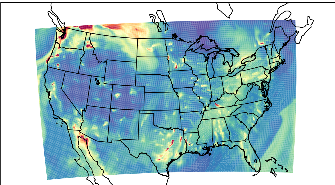
WRF 2019-11-03_04:00:00
