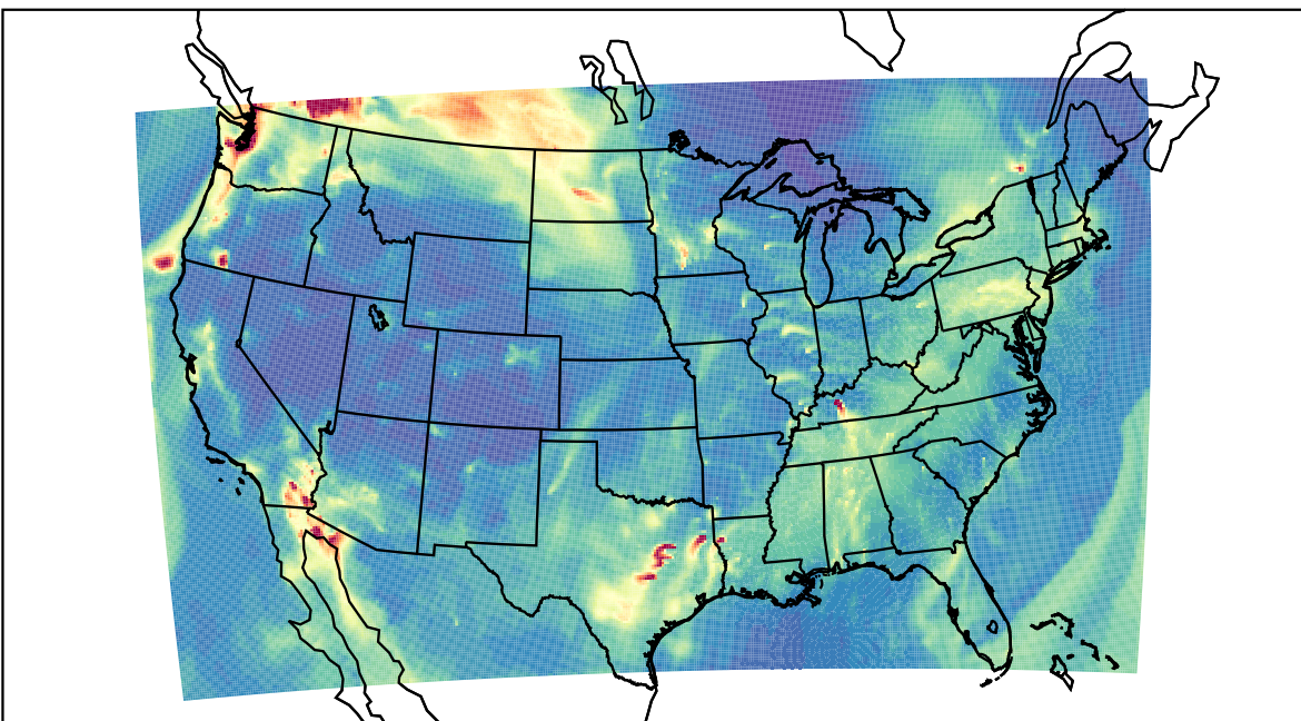
WRF 2019-11-03_08:00:00
