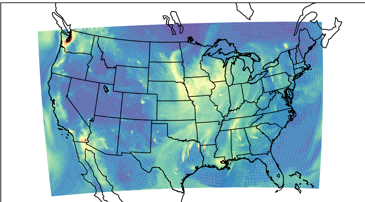
WRF 2019-11-04_16:00:00
