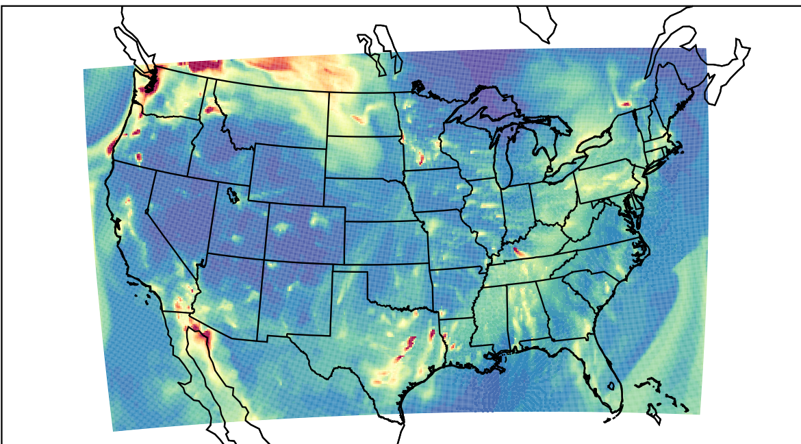
WRF 2019-11-03_05:00:00
