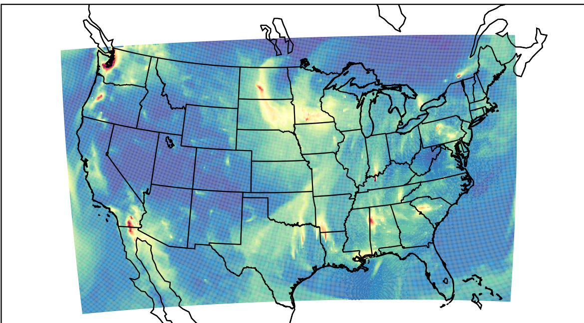
WRF 2019-11-04_09:00:00
