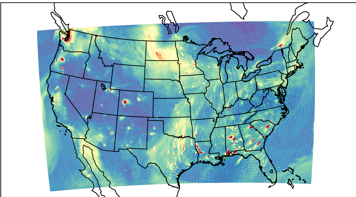
WRF 2019-11-04_01:00:00
