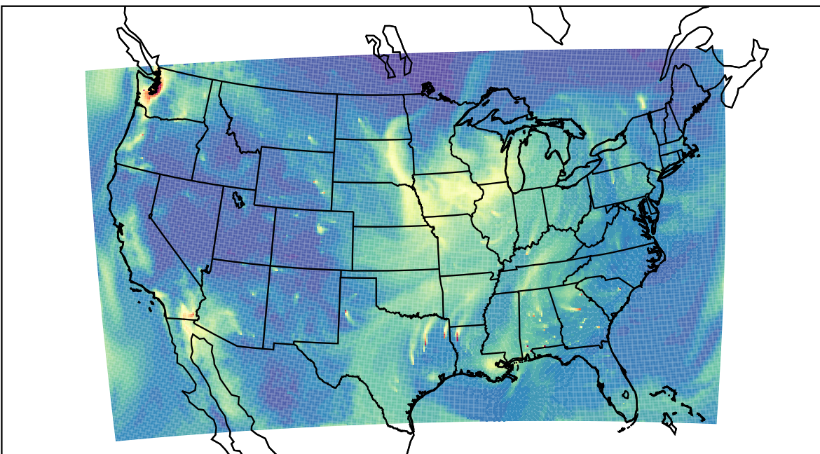
WRF 2019-11-04_17:00:00
