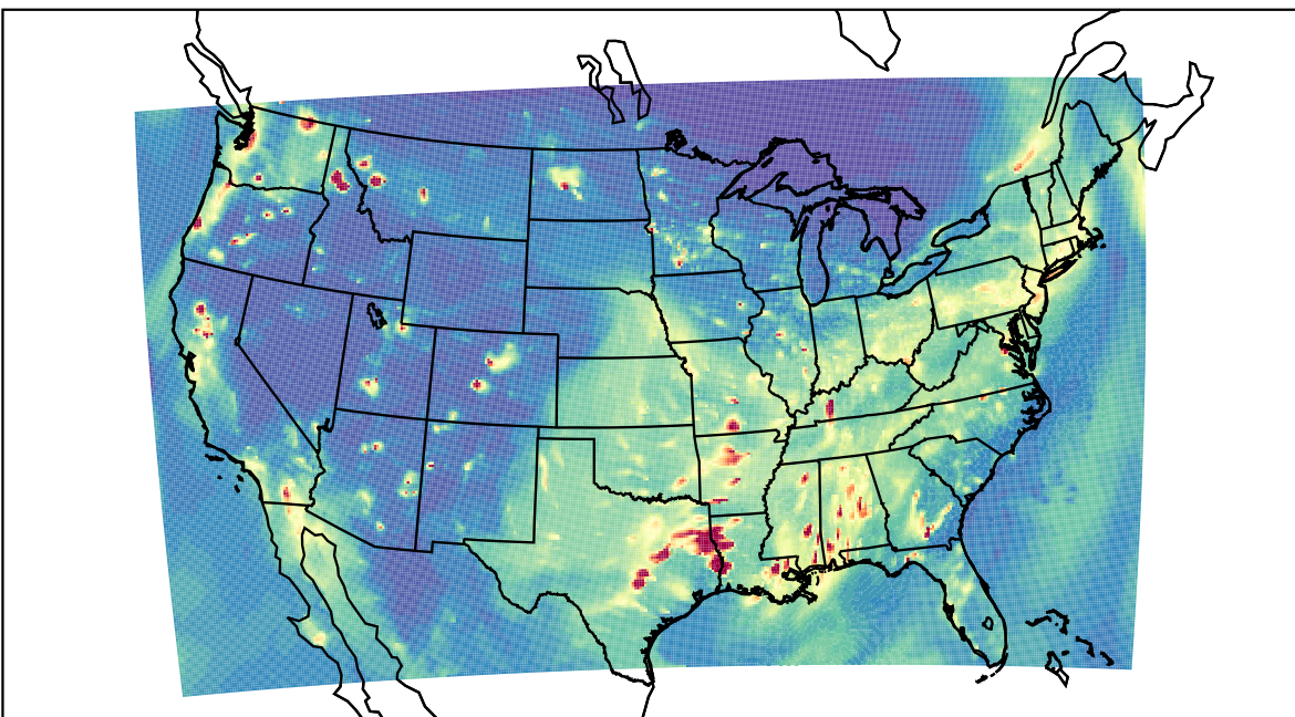
WRF 2019-11-06_03:00:00
