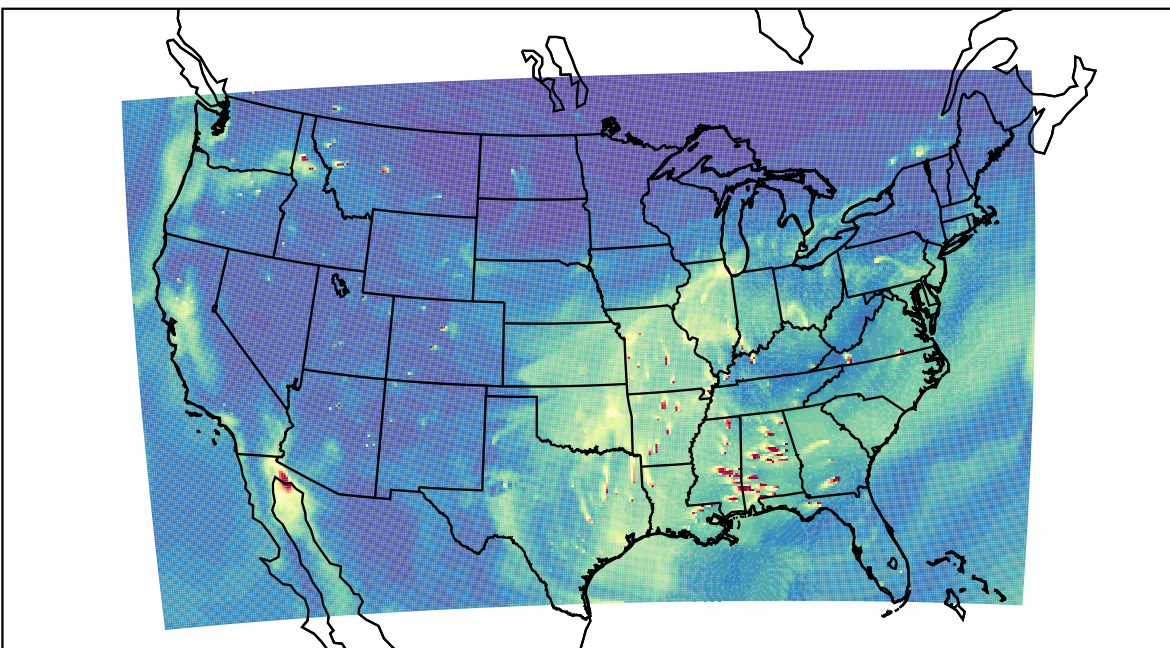
WRF 2019-11-06_21:00:00
