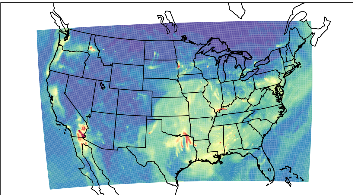
WRF 2019-11-06_13:00:00
