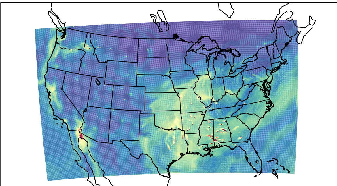
WRF 2019-11-06_19:00:00
