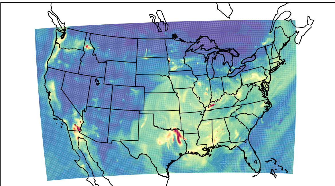
WRF 2019-11-06_10:00:00
