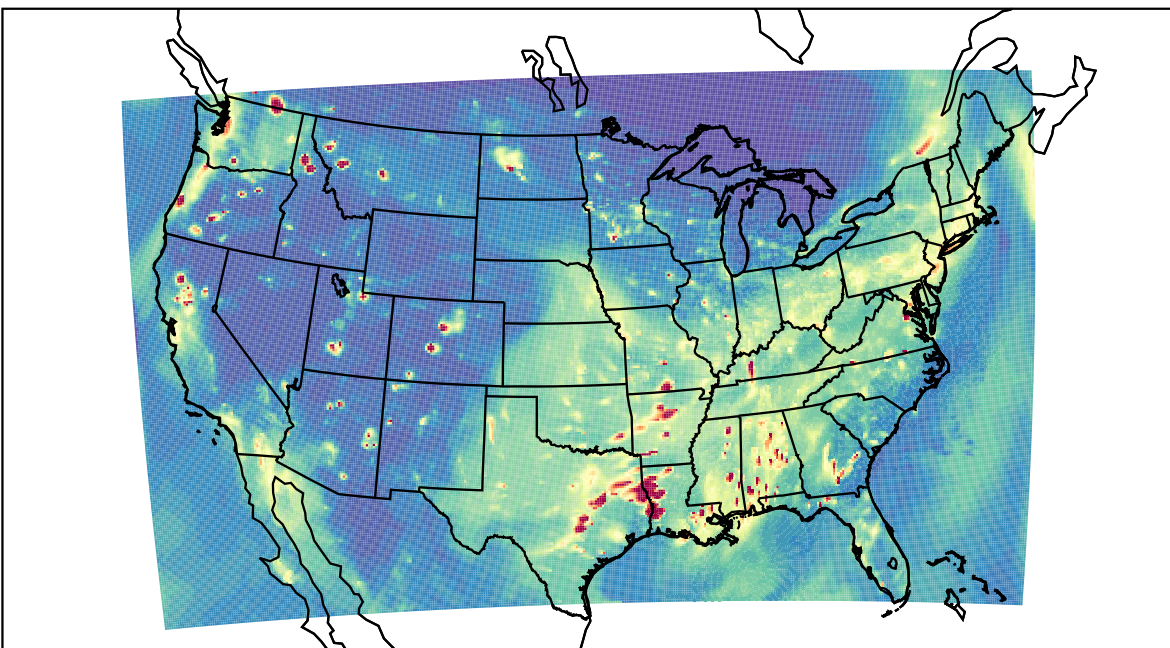
WRF 2019-11-06_02:00:00
