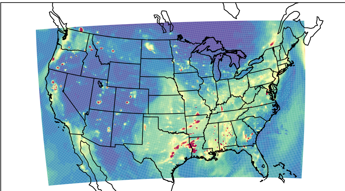
WRF 2019-11-06_01:00:00
