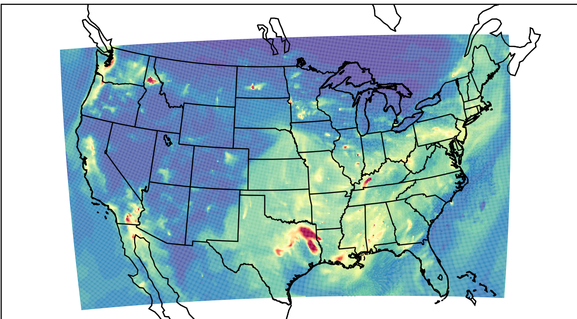
WRF 2019-11-06_07:00:00
