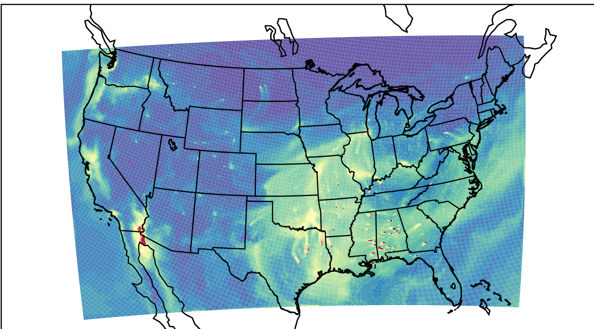
WRF 2019-11-06_18:00:00
