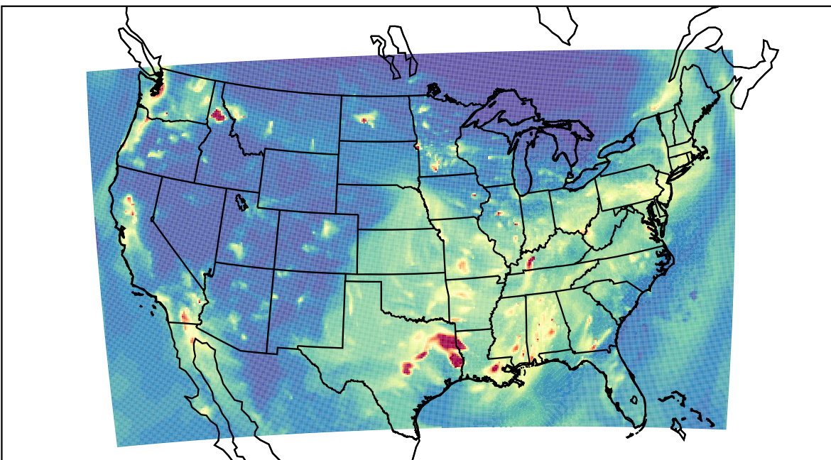
WRF 2019-11-06_05:00:00
