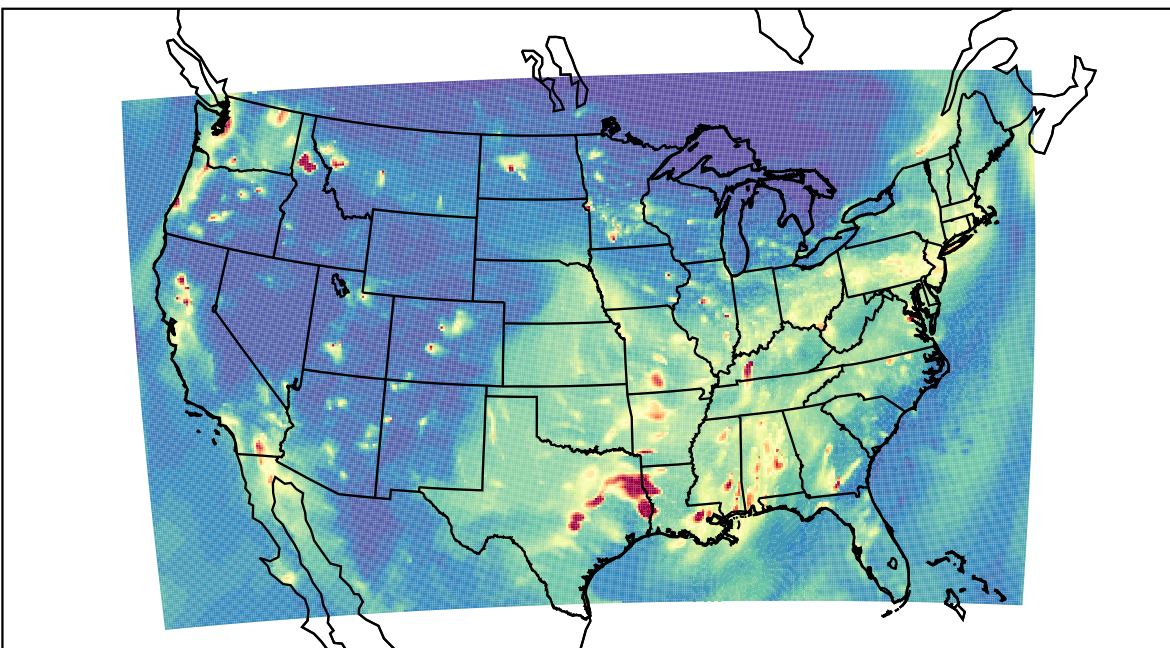
WRF 2019-11-06_04:00:00
