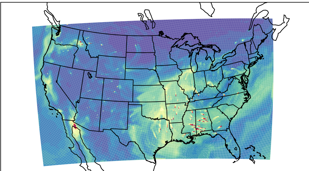
WRF 2019-11-06_20:00:00
