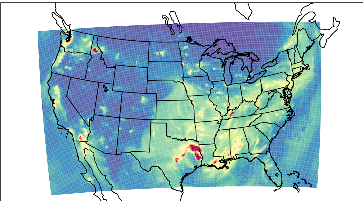
WRF 2019-11-06_06:00:00
