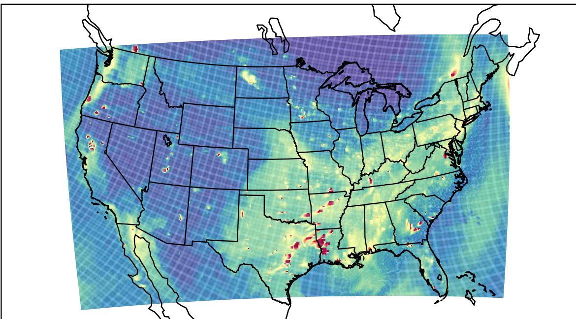
WRF 2019-11-06_00:00:00
