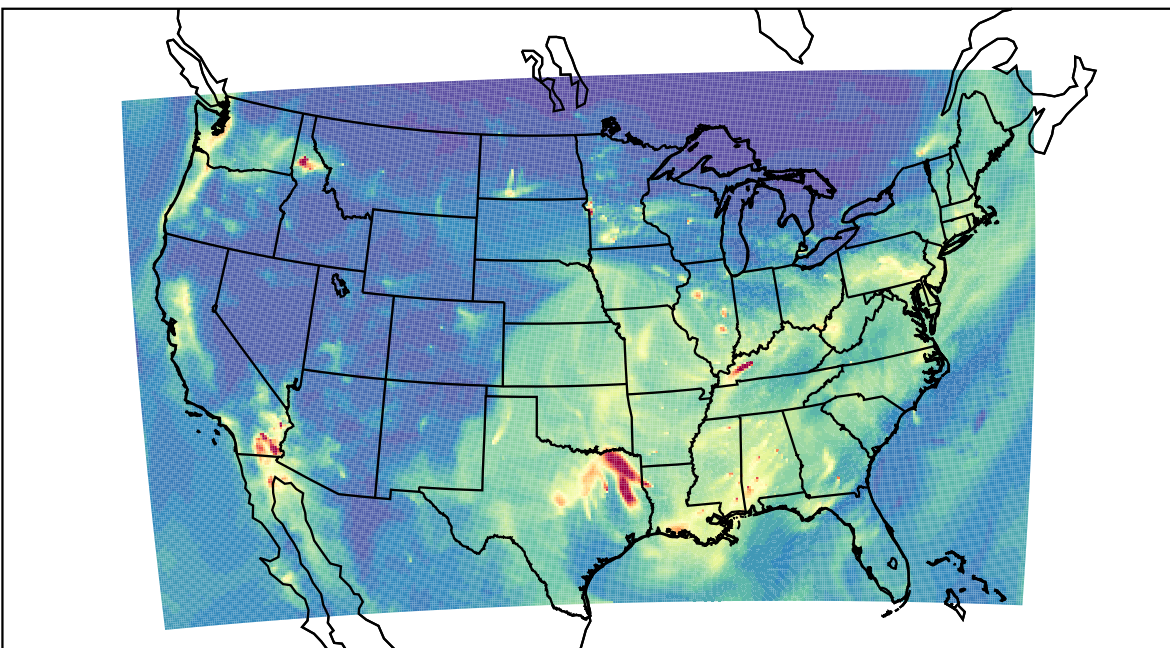
WRF 2019-11-06_09:00:00
