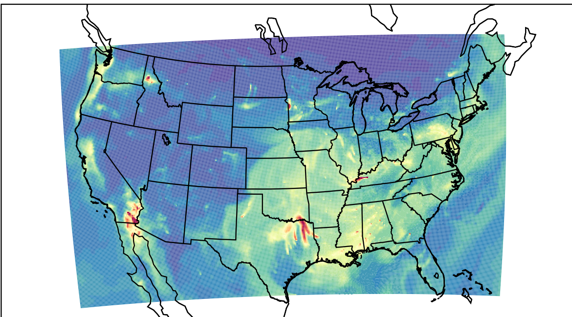
WRF 2019-11-06_12:00:00
