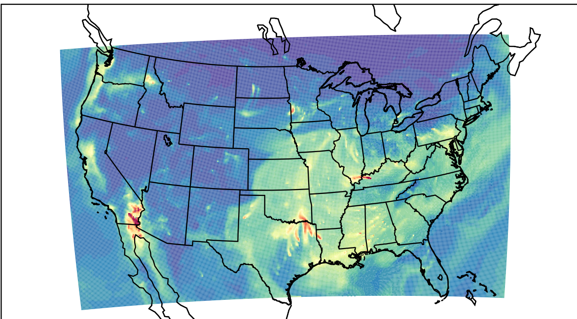
WRF 2019-11-06_14:00:00
