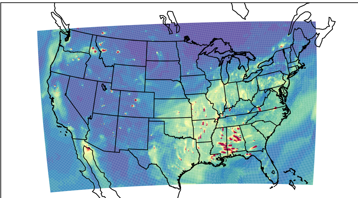
WRF 2019-11-06_23:00:00
