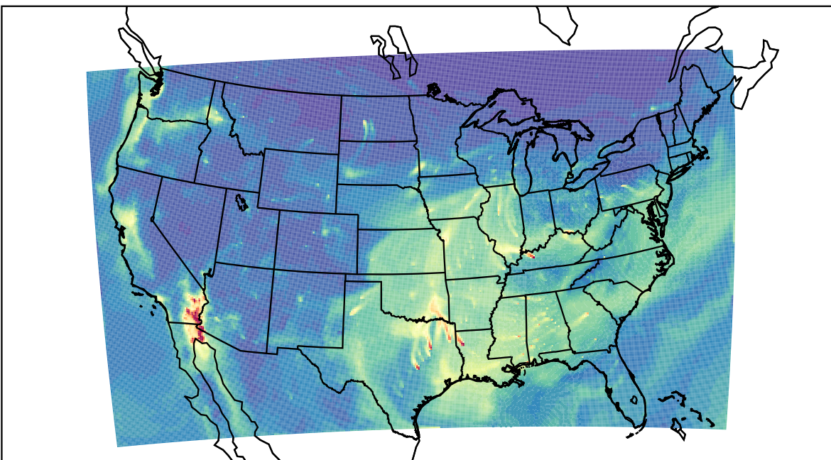
WRF 2019-11-06_16:00:00
