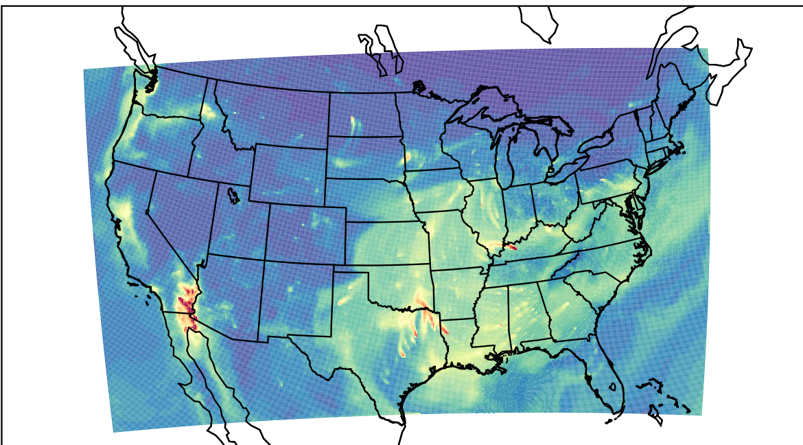
WRF 2019-11-06_15:00:00
