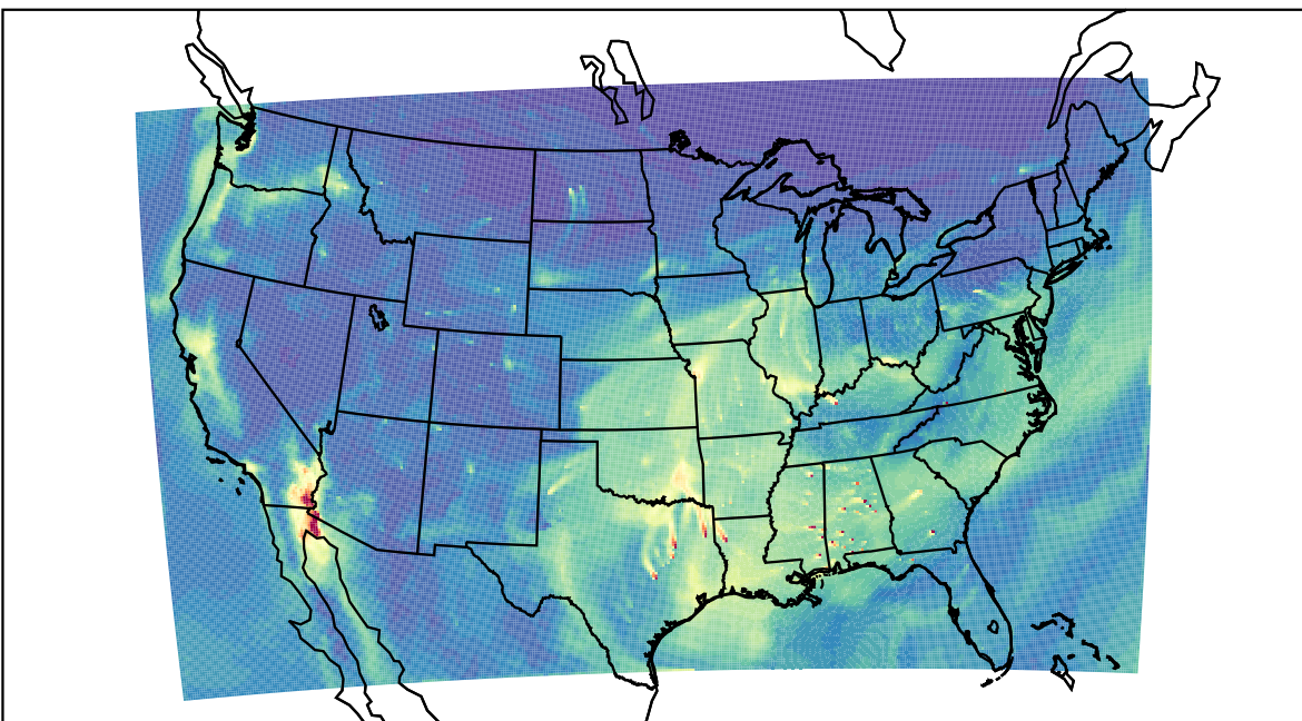
WRF 2019-11-06_17:00:00
