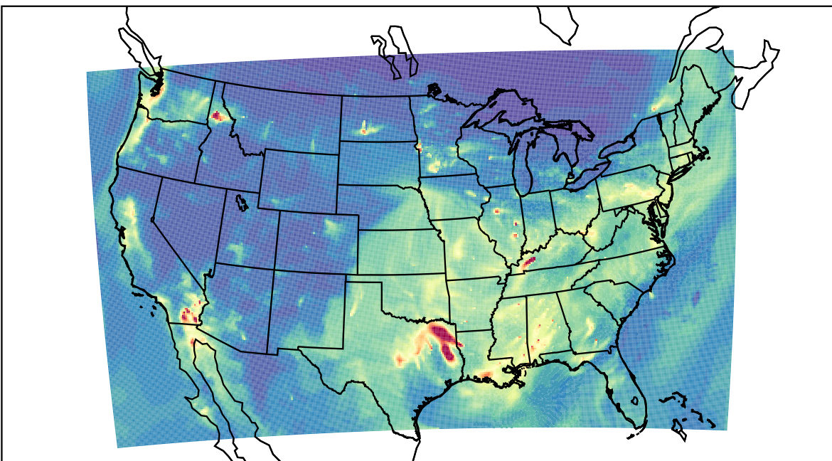
WRF 2019-11-06_08:00:00
