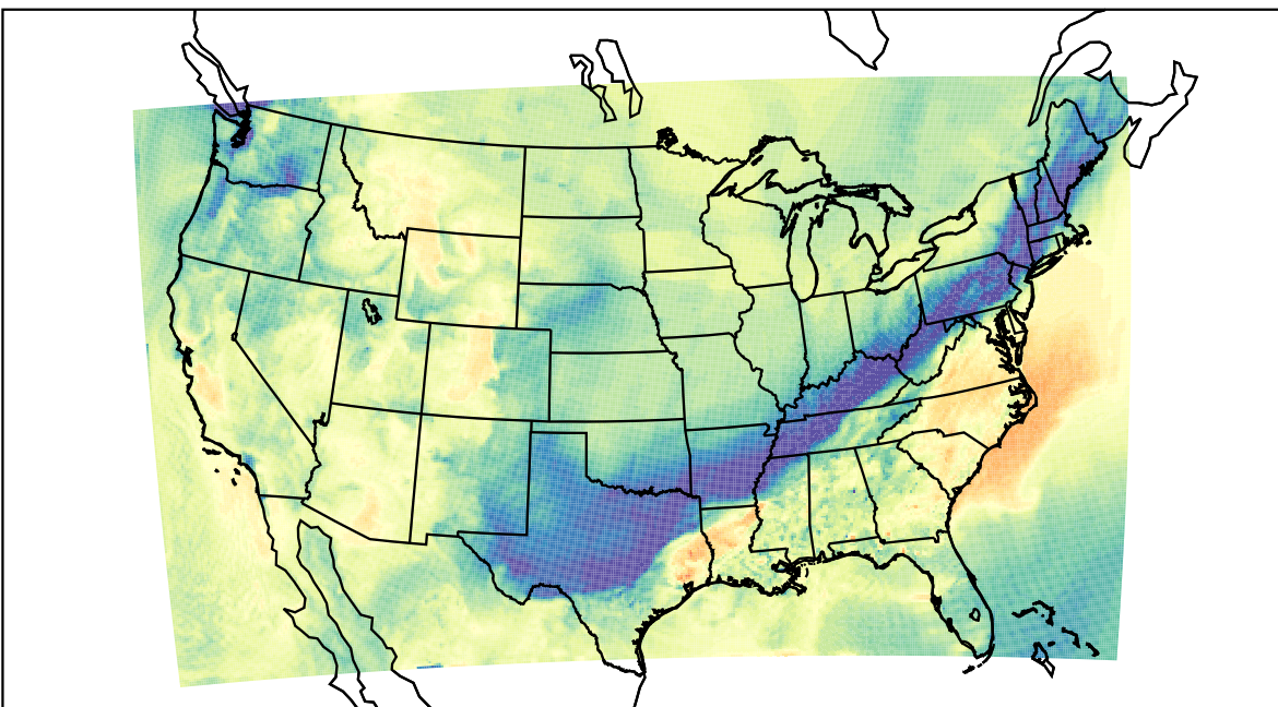
WRF (2019-11-07_20:00:00)
