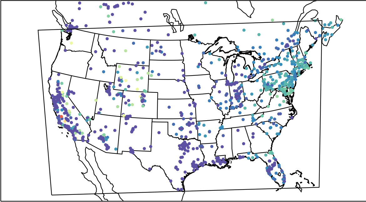
AirNOW (2019-11-08_14:00:00)
