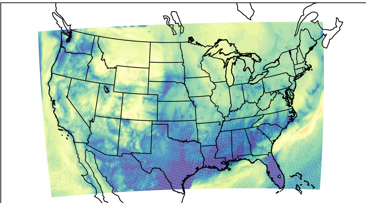
WRF (2019-11-08_13:00:00)
