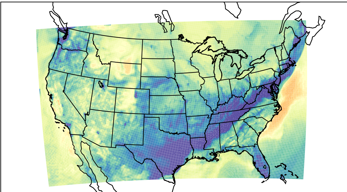
WRF (2019-11-08_03:00:00)
