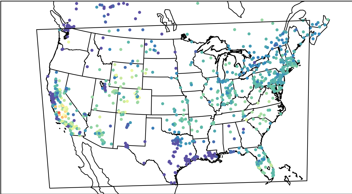
AirNOW (2019-11-08_18:00:00)
