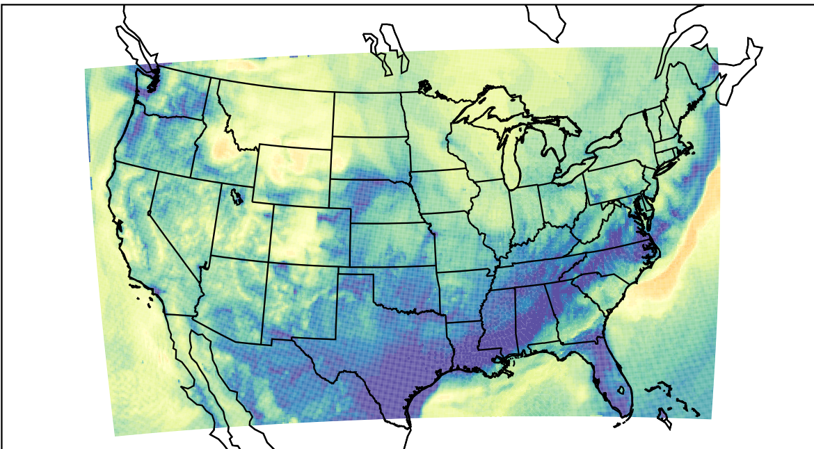
WRF (2019-11-08_09:00:00)
