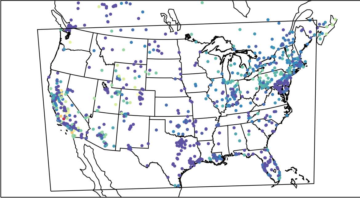
AirNOW (2019-11-08_03:00:00)
