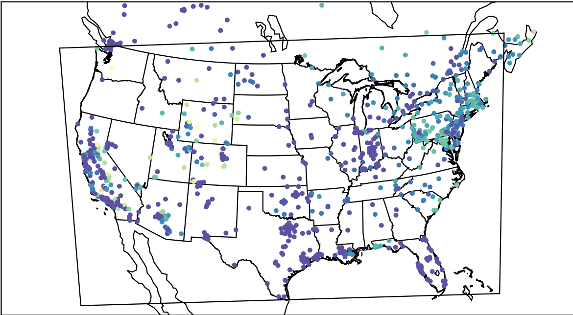
AirNOW (2019-11-08_10:00:00)
