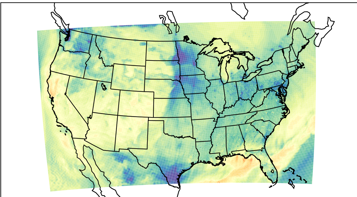
WRF (2019-11-08_22:00:00)
