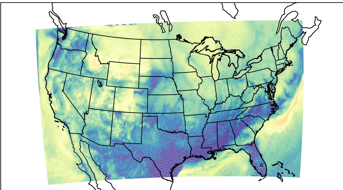
WRF (2019-11-08_11:00:00)
