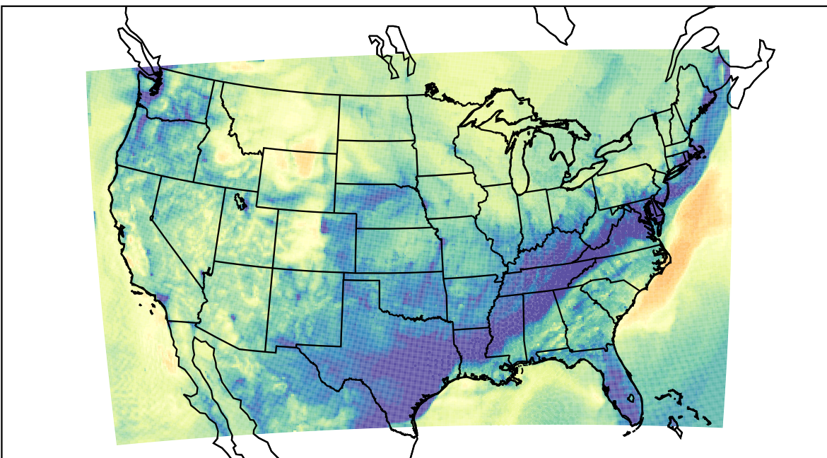
WRF (2019-11-08_04:00:00)
