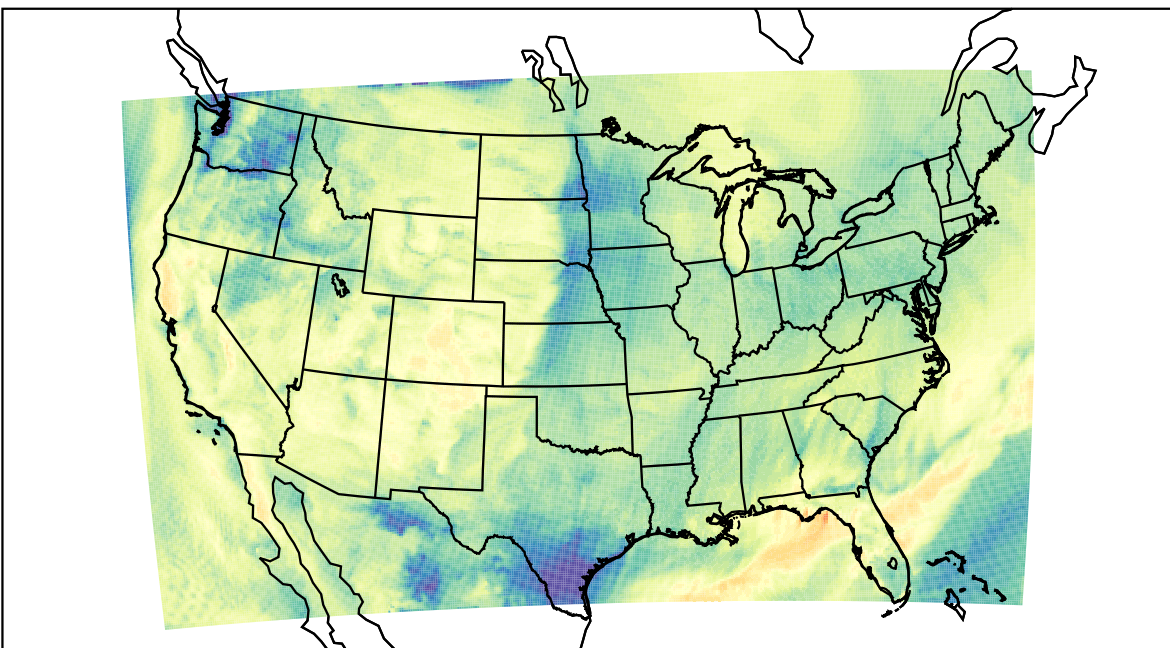
WRF (2019-11-08_20:00:00)
