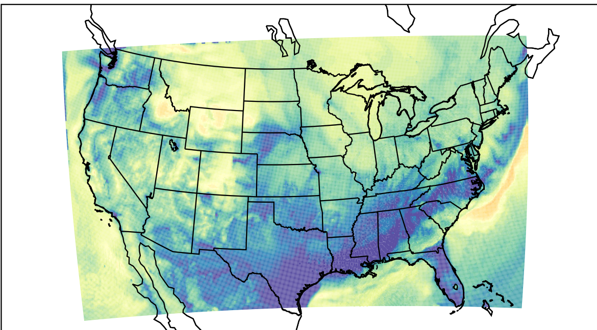
WRF (2019-11-08_10:00:00)
