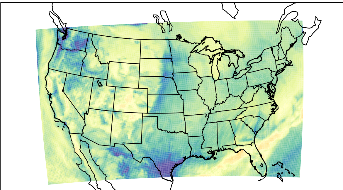
WRF (2019-11-08_18:00:00)
