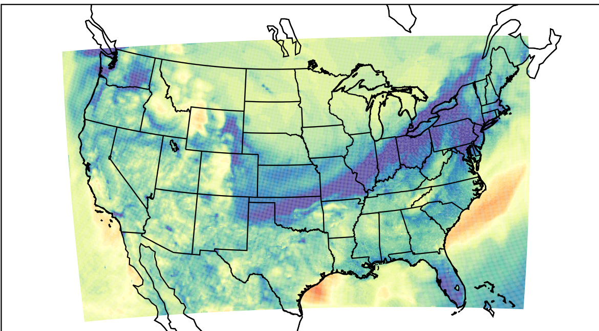
WRF (2019-11-07_06:00:00)
