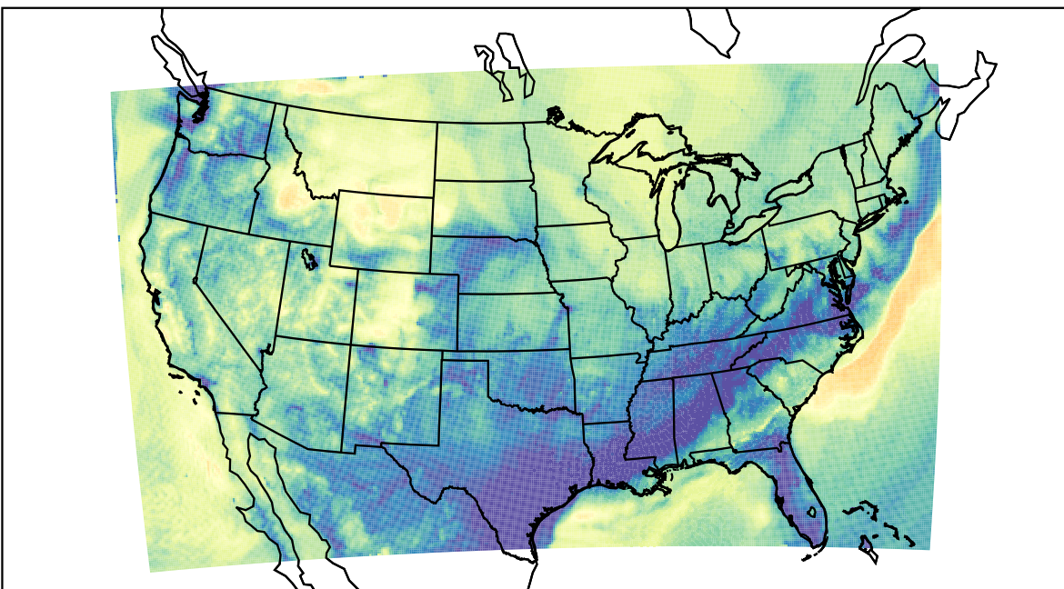
WRF (2019-11-08_08:00:00)
