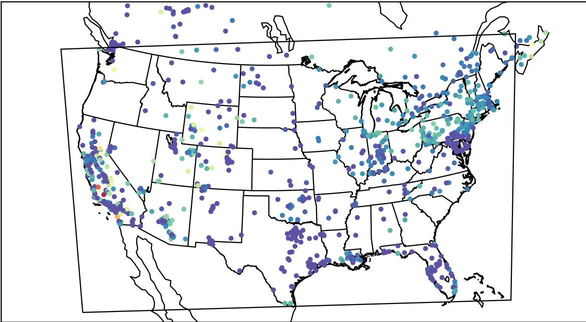
AirNOW (2019-11-08_04:00:00)
