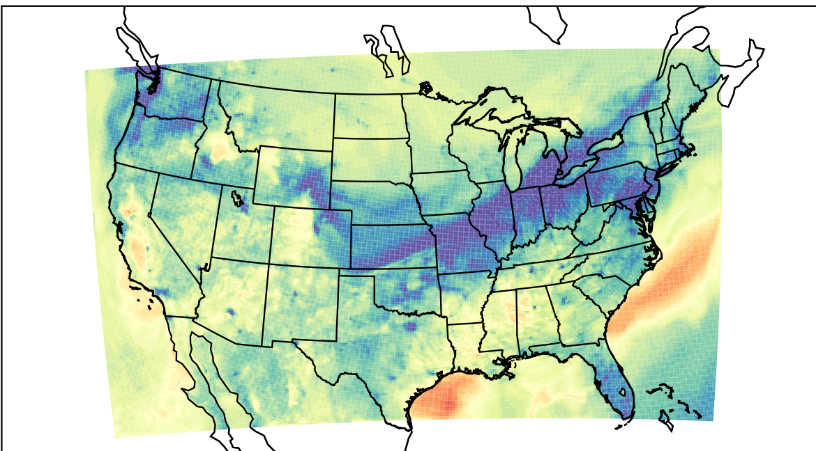
WRF (2019-11-07_01:00:00)
