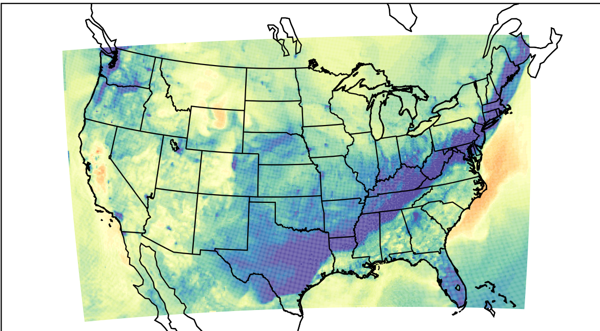
WRF (2019-11-08_01:00:00)
