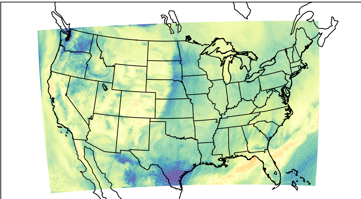
WRF (2019-11-08_19:00:00)
