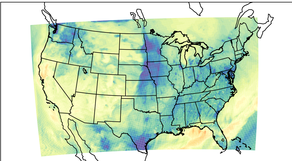
WRF (2019-11-08_23:00:00)
