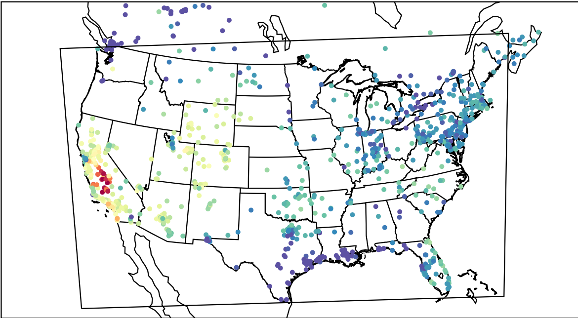
AirNOW (2019-11-08_22:00:00)
