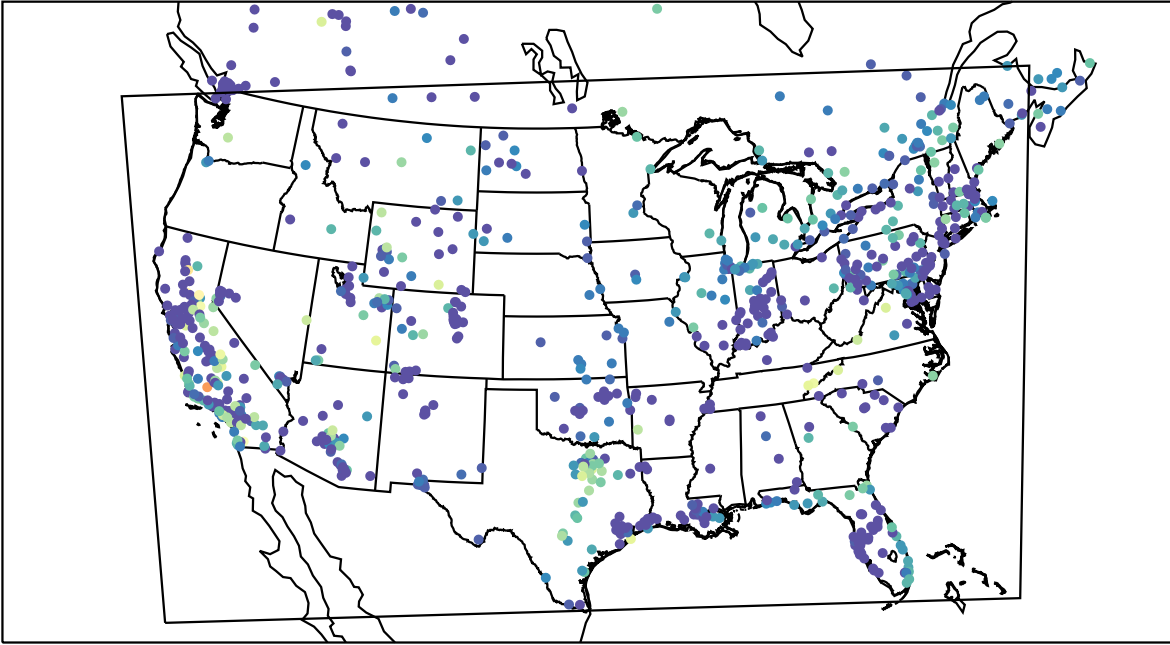
AirNOW (2019-11-07_08:00:00)
