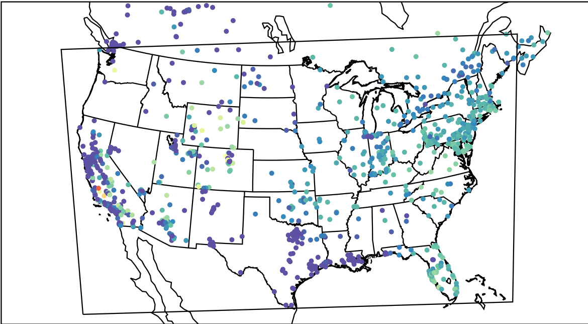
AirNOW (2019-11-08_16:00:00)
