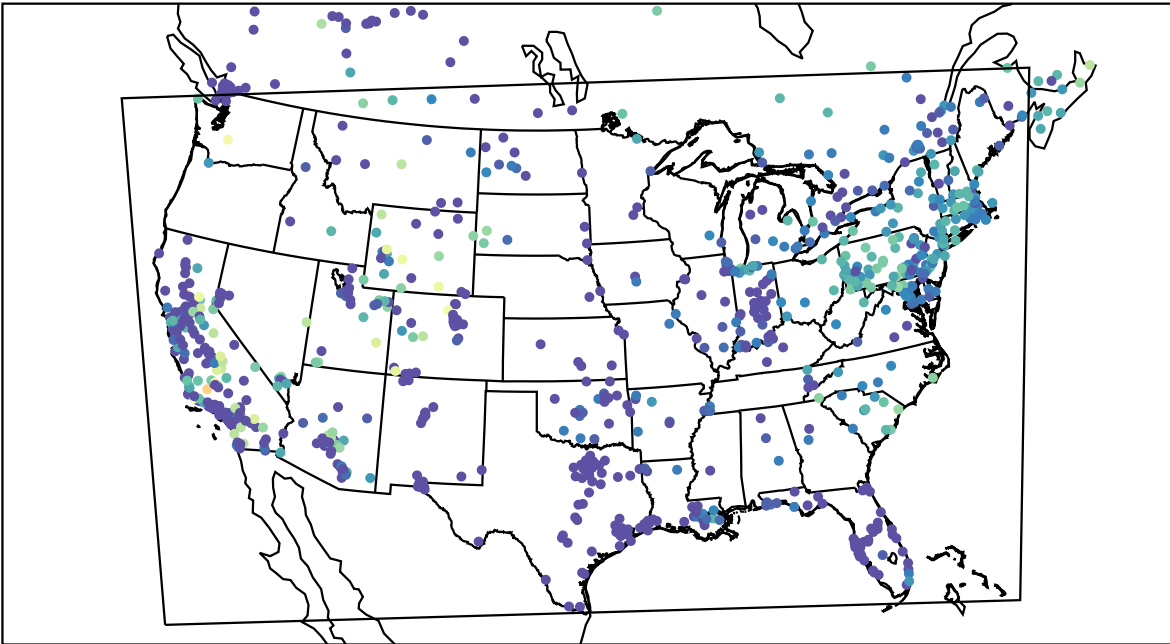
AirNOW (2019-11-08_08:00:00)
