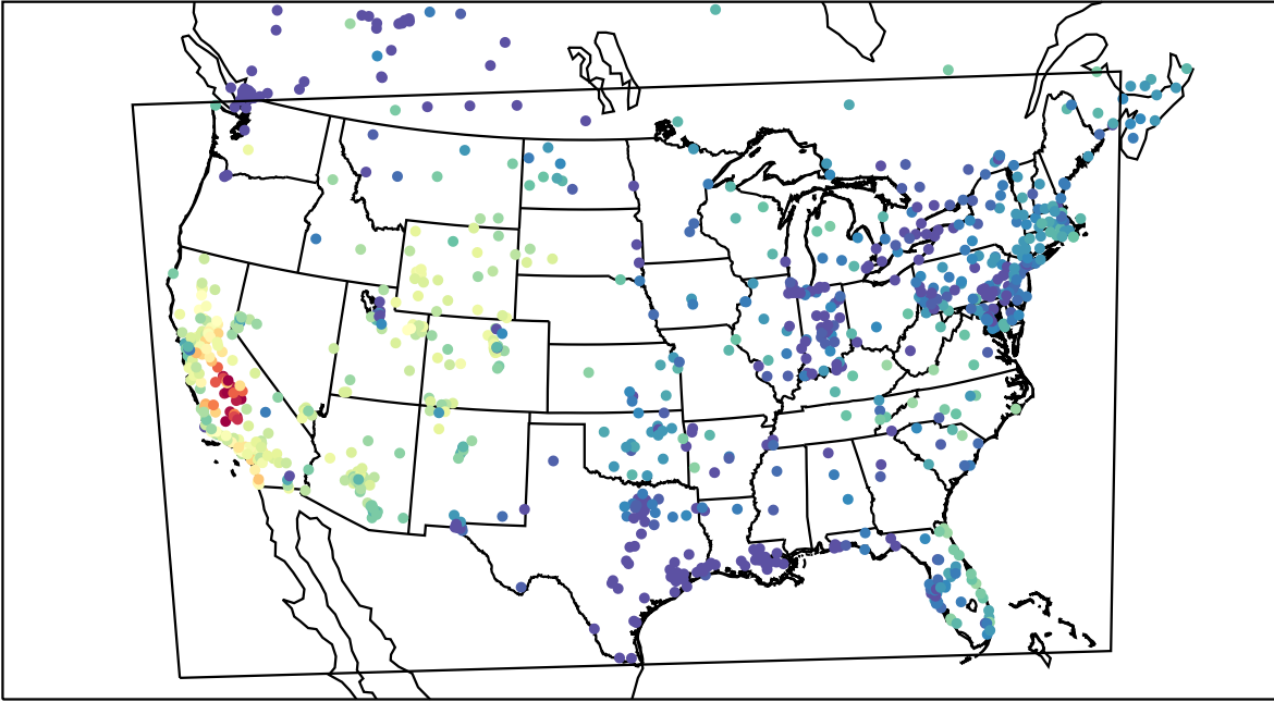
AirNOW (2019-11-08_23:00:00)
