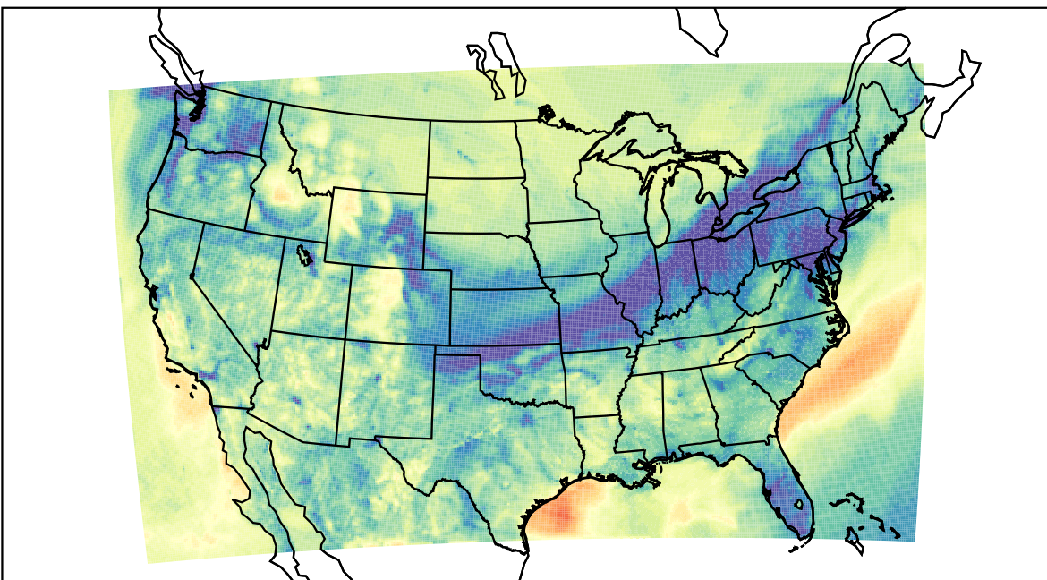
WRF (2019-11-07_04:00:00)
