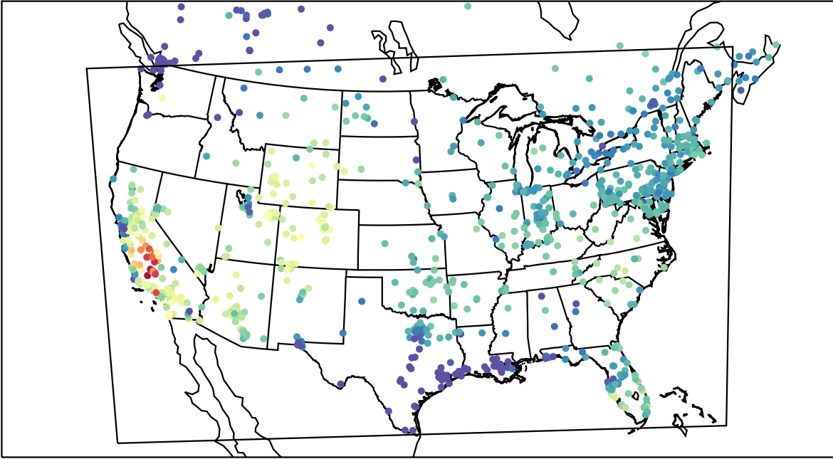
AirNOW (2019-11-08_20:00:00)
