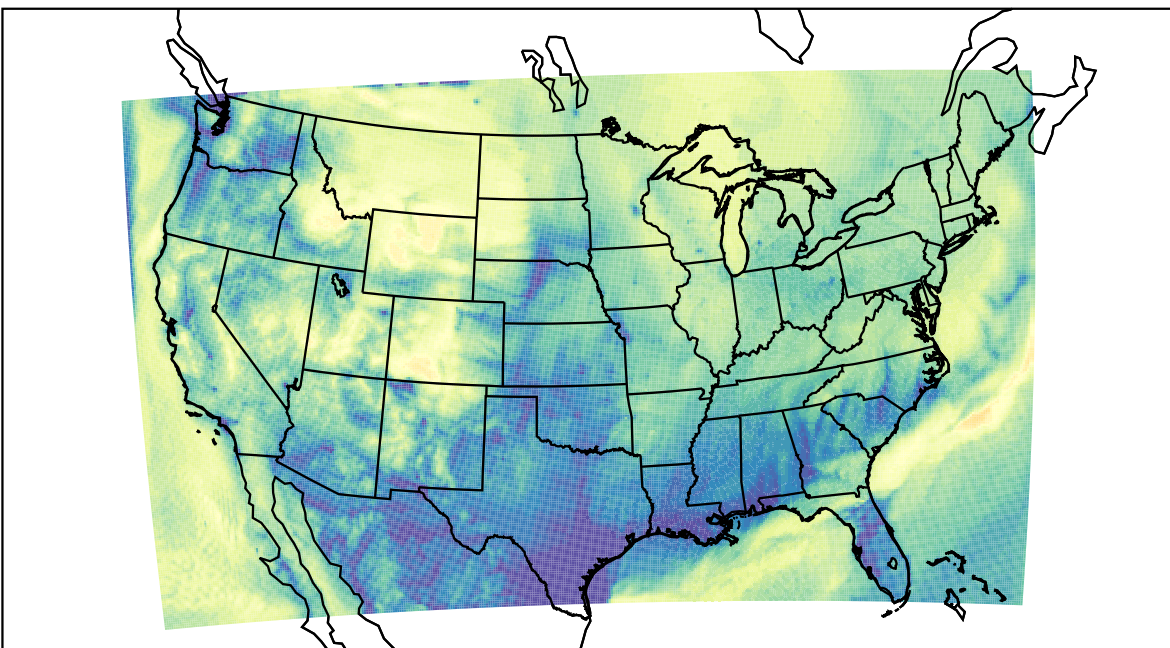
WRF (2019-11-08_14:00:00)
