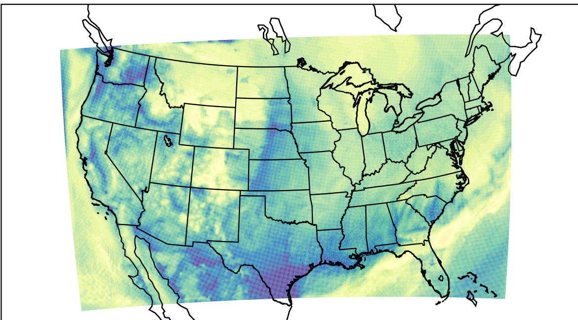
WRF (2019-11-08_16:00:00)
