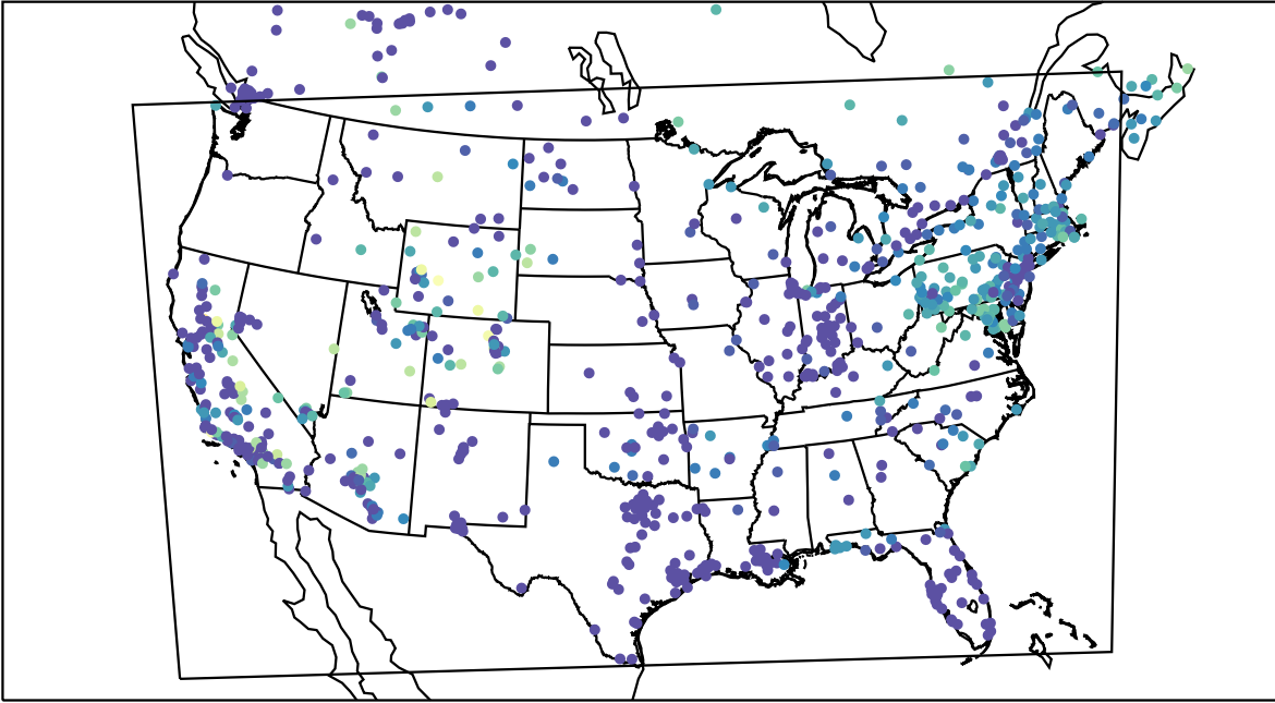
AirNOW (2019-11-08_11:00:00)
