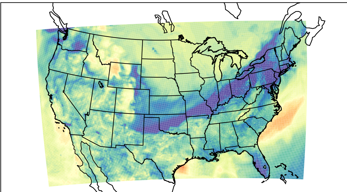
WRF (2019-11-07_08:00:00)
