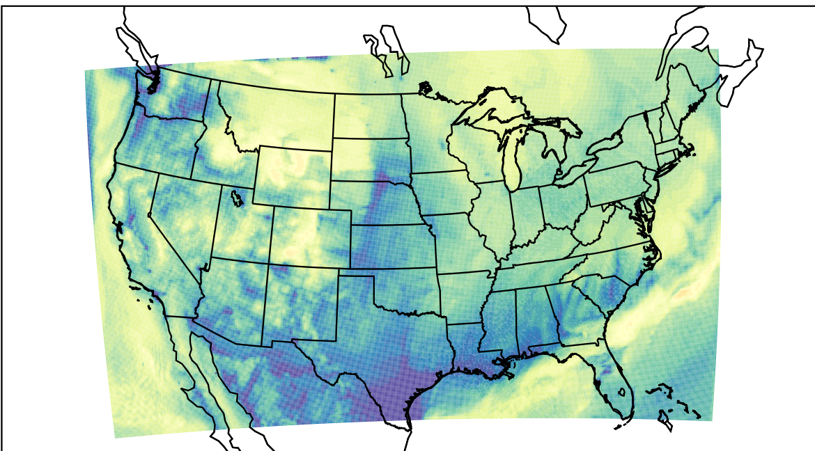
WRF (2019-11-08_15:00:00)
