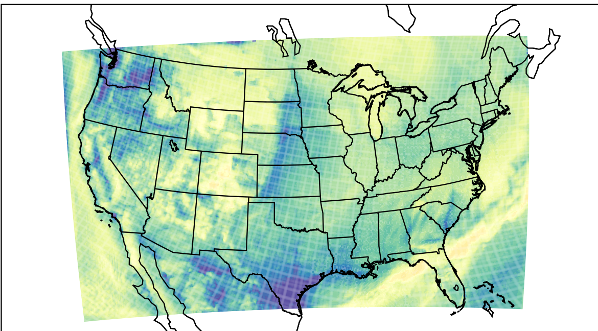
WRF (2019-11-08_17:00:00)
