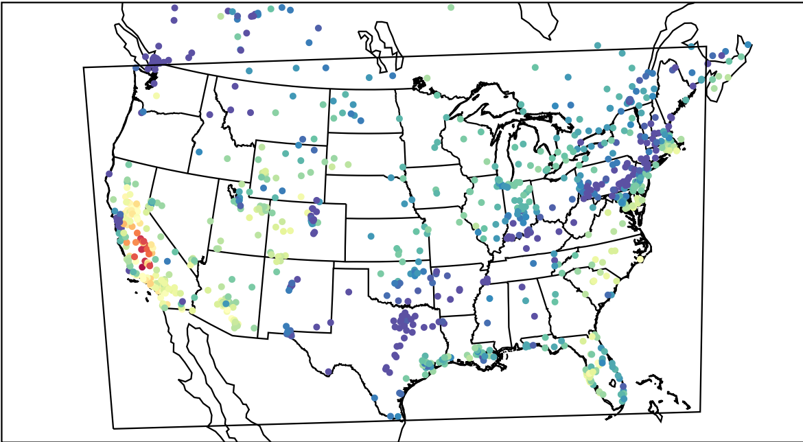
AirNOW (2019-11-07_20:00:00)
