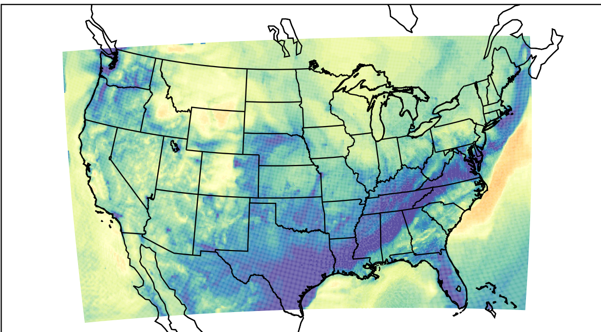
WRF (2019-11-08_06:00:00)
