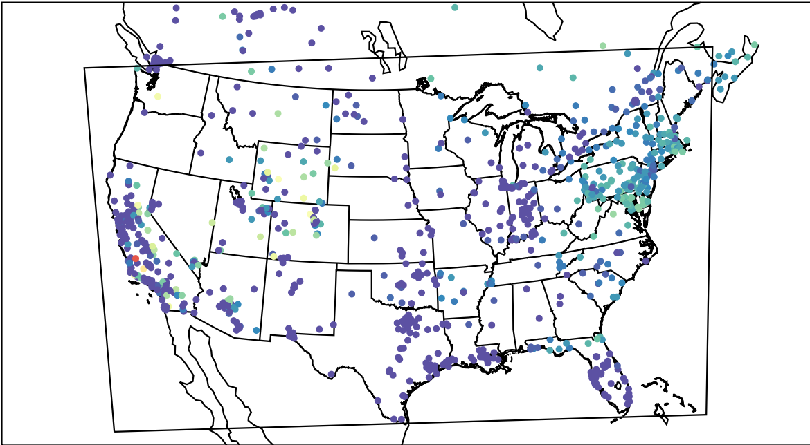
AirNOW (2019-11-08_13:00:00)
