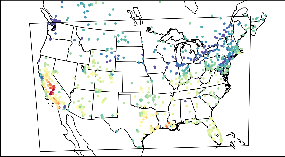
AirNOW (2019-11-10_21:00:00)
