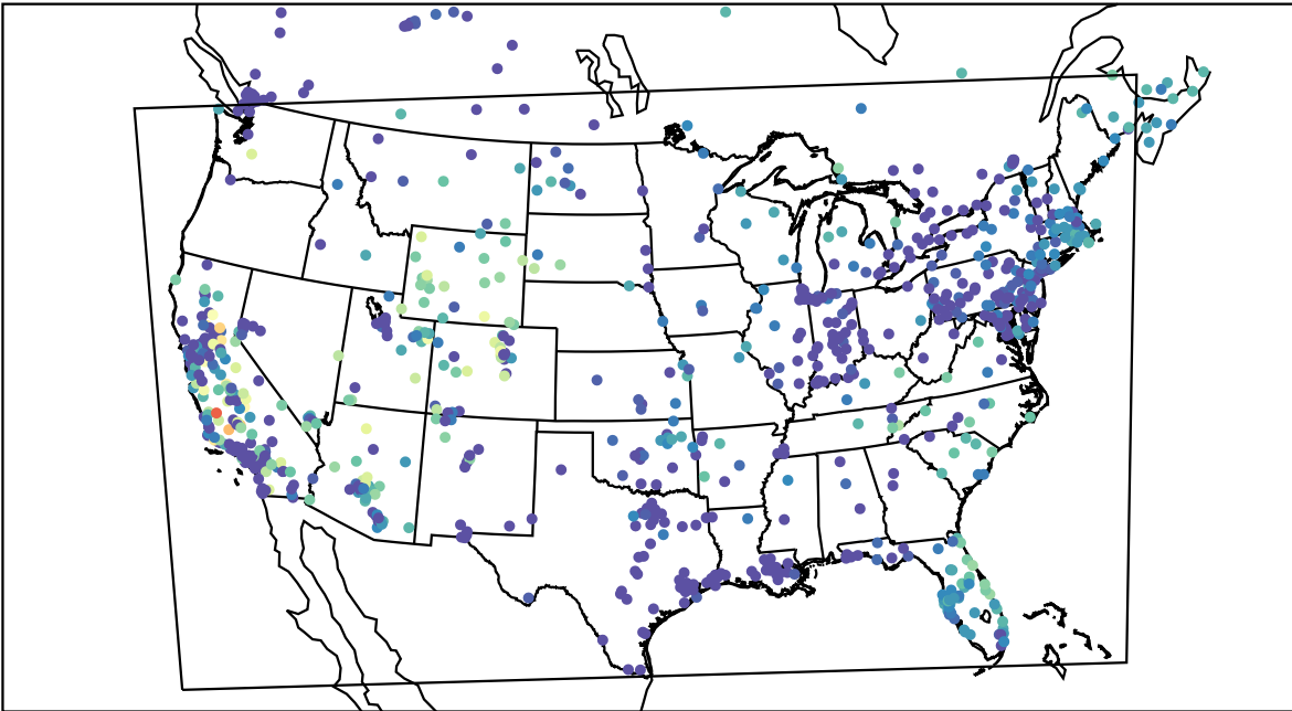
AirNOW (2019-11-09_03:00:00)
