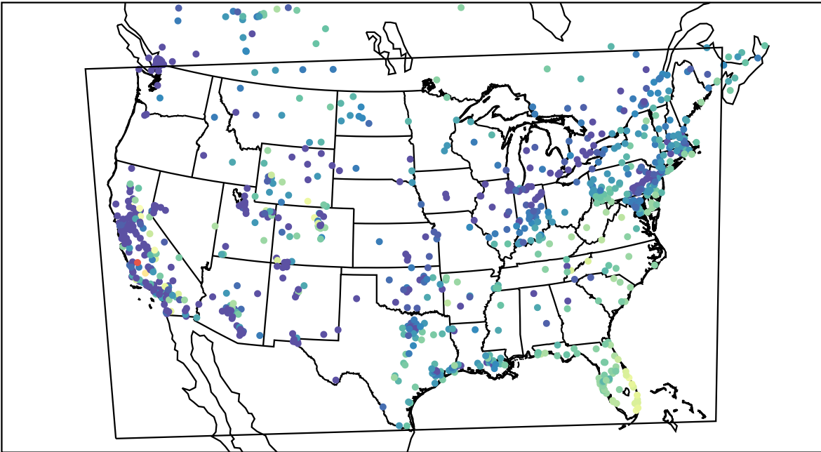
AirNOW (2019-11-10_15:00:00)
