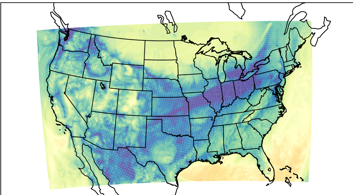
WRF (2019-11-10_15:00:00)
