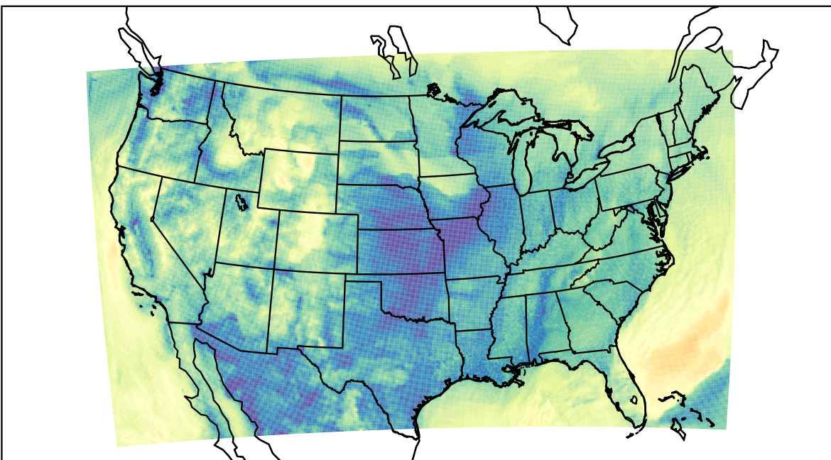
WRF (2019-11-09_15:00:00)
