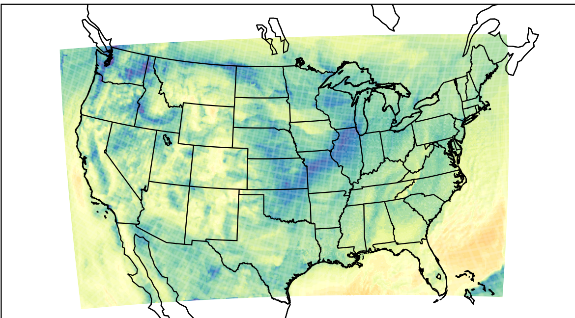
WRF (2019-11-09_18:00:00)
