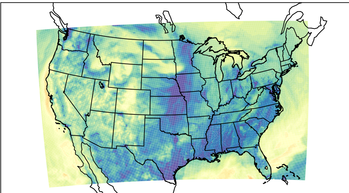
WRF (2019-11-09_06:00:00)
