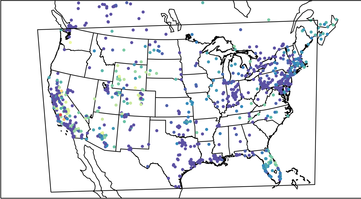
AirNOW (2019-11-09_04:00:00)
