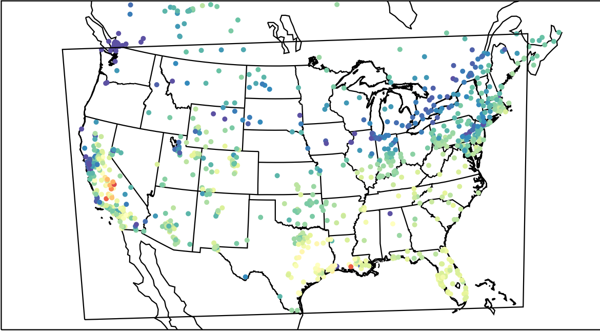
AirNOW (2019-11-10_18:00:00)
