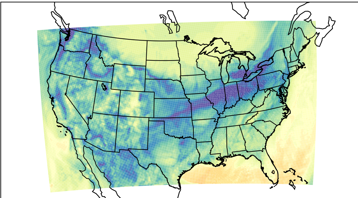
WRF (2019-11-10_16:00:00)
