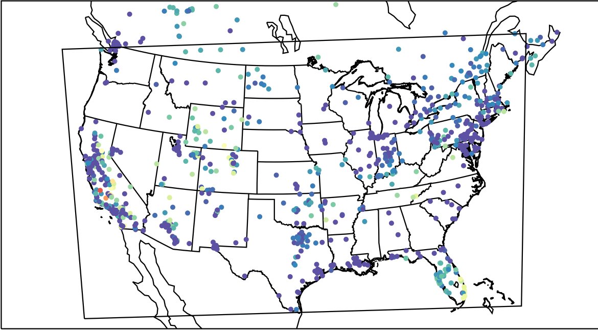
AirNOW (2019-11-10_07:00:00)
