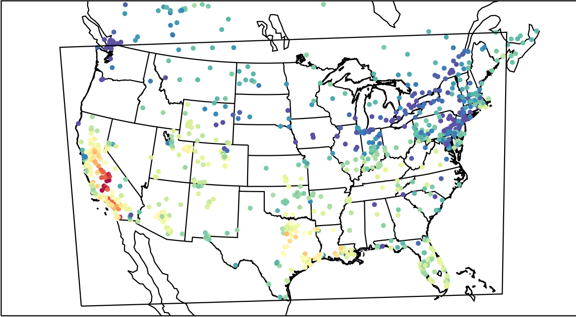
AirNOW (2019-11-10_22:00:00)
