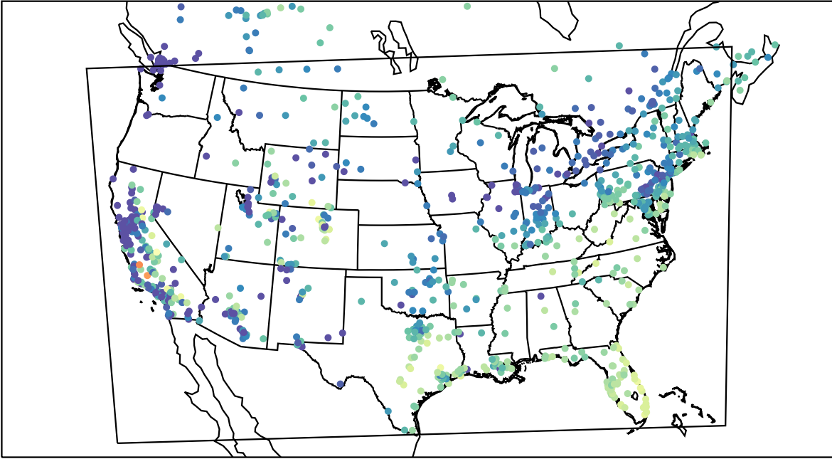
AirNOW (2019-11-10_16:00:00)
