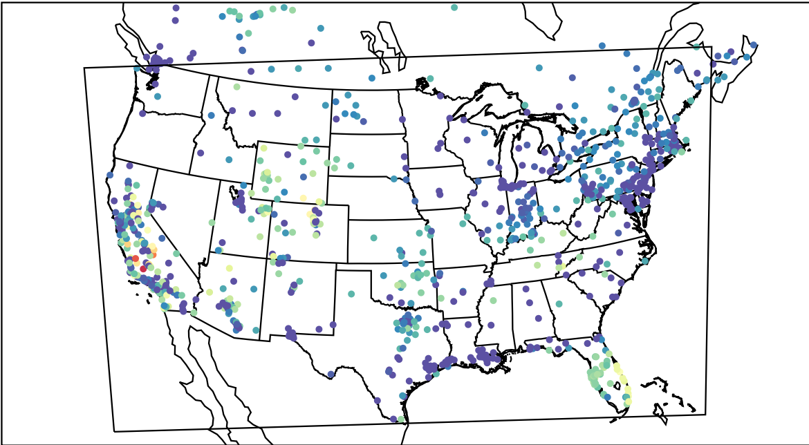
AirNOW (2019-11-10_02:00:00)
