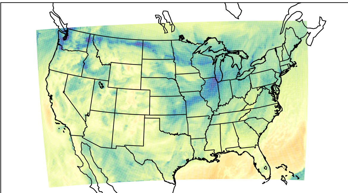
WRF (2019-11-09_20:00:00)
