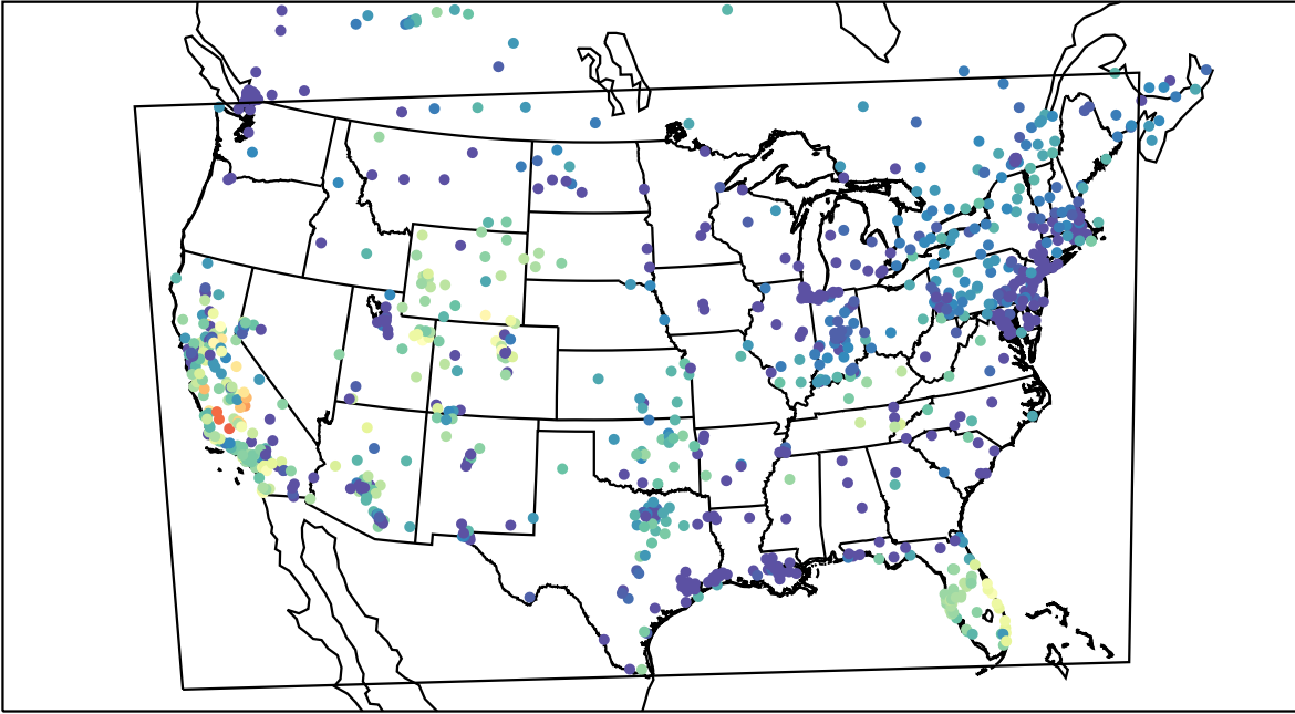
AirNOW (2019-11-10_01:00:00)
