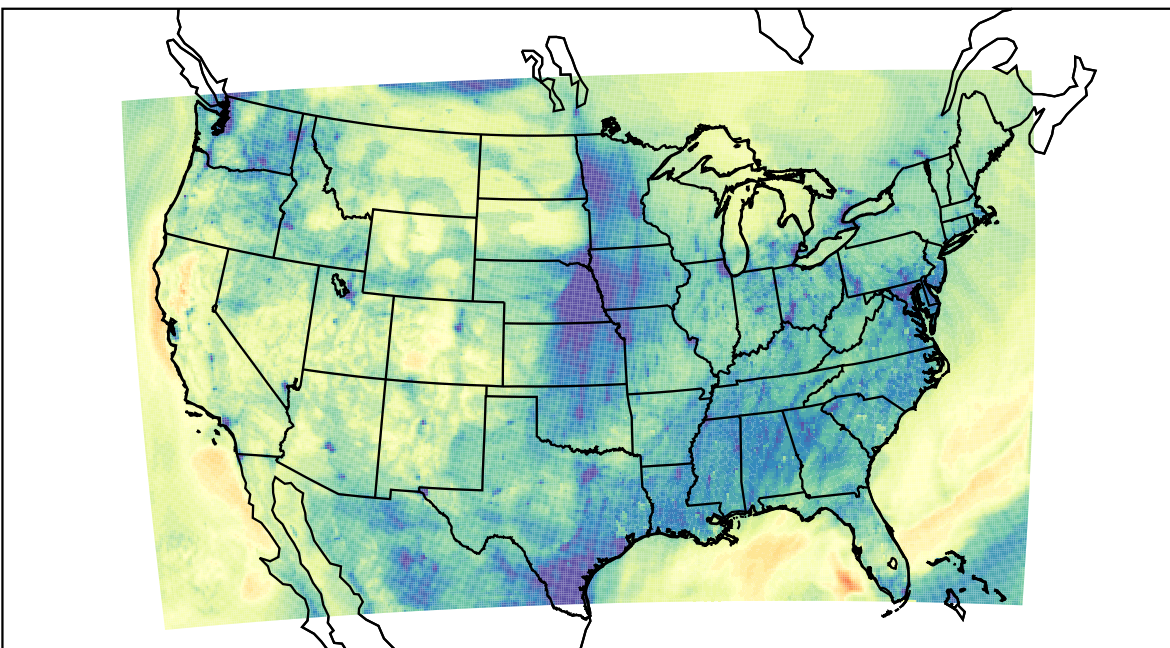
WRF (2019-11-09_01:00:00)
