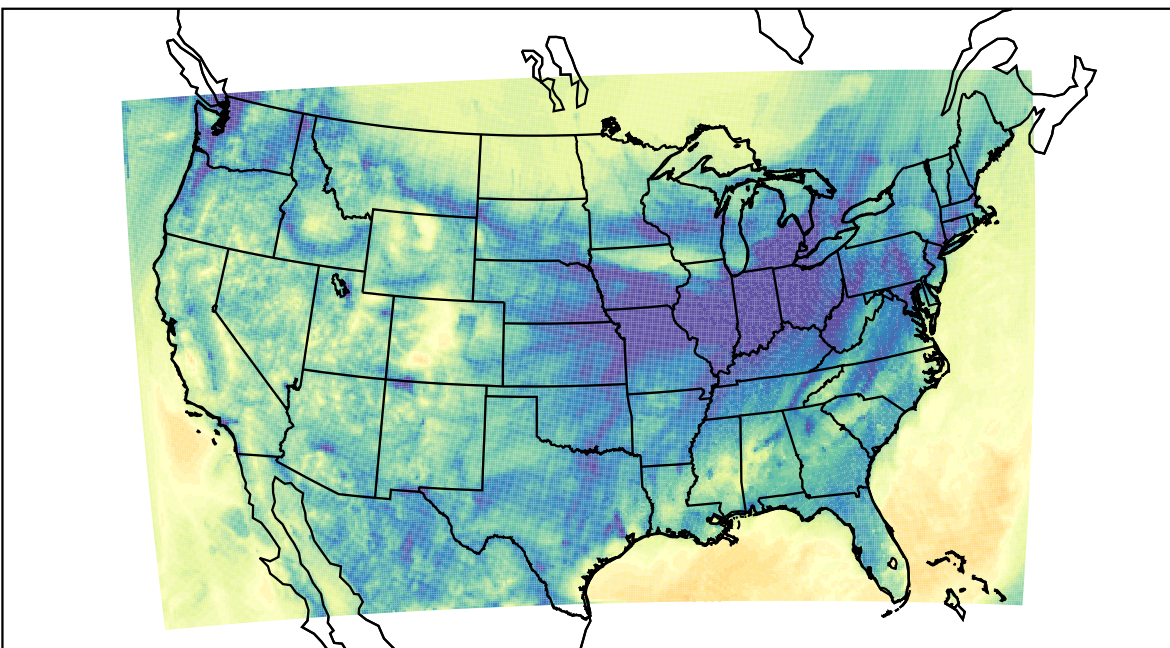
WRF (2019-11-10_07:00:00)
