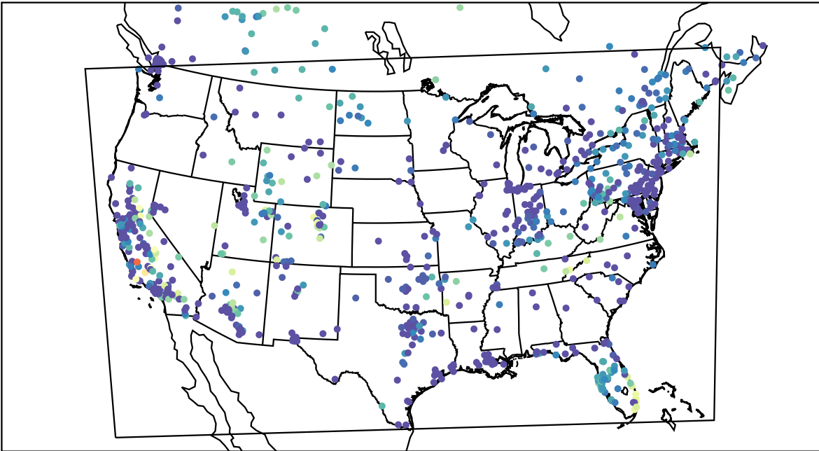
AirNOW (2019-11-10_09:00:00)
