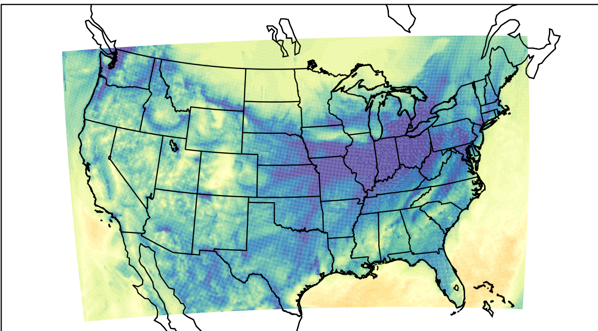
WRF (2019-11-10_09:00:00)
