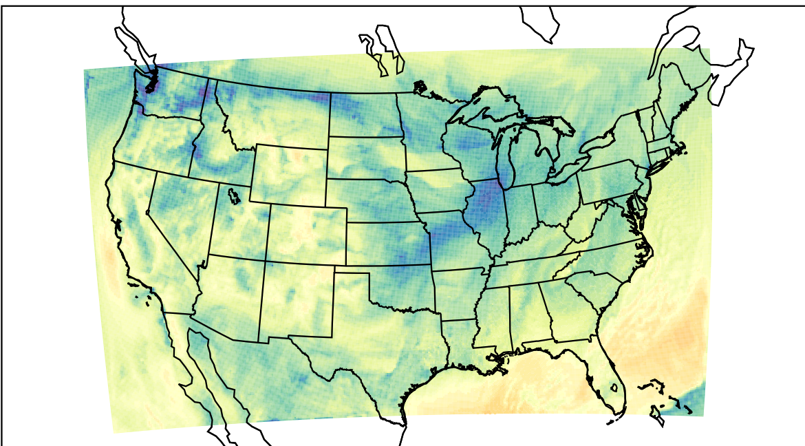
WRF (2019-11-09_19:00:00)
