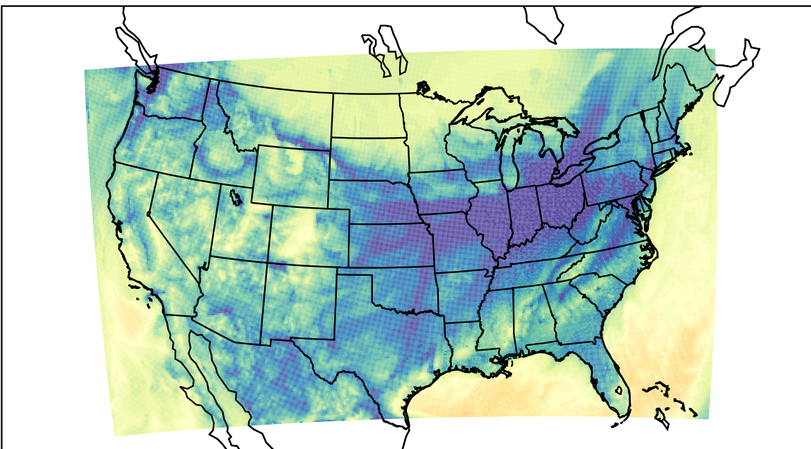
WRF (2019-11-10_11:00:00)
