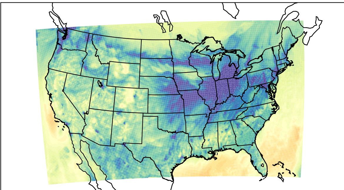
WRF (2019-11-10_02:00:00)
