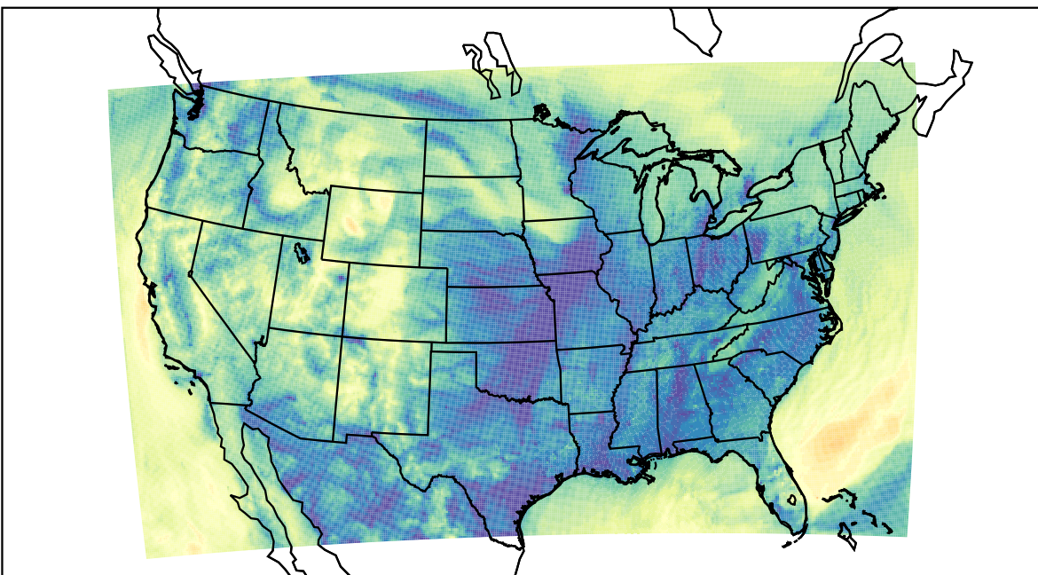
WRF (2019-11-09_13:00:00)
