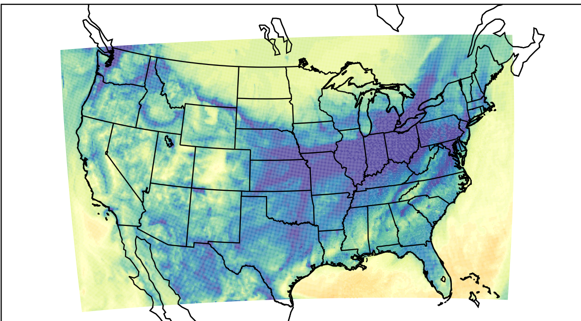
WRF (2019-11-10_12:00:00)
