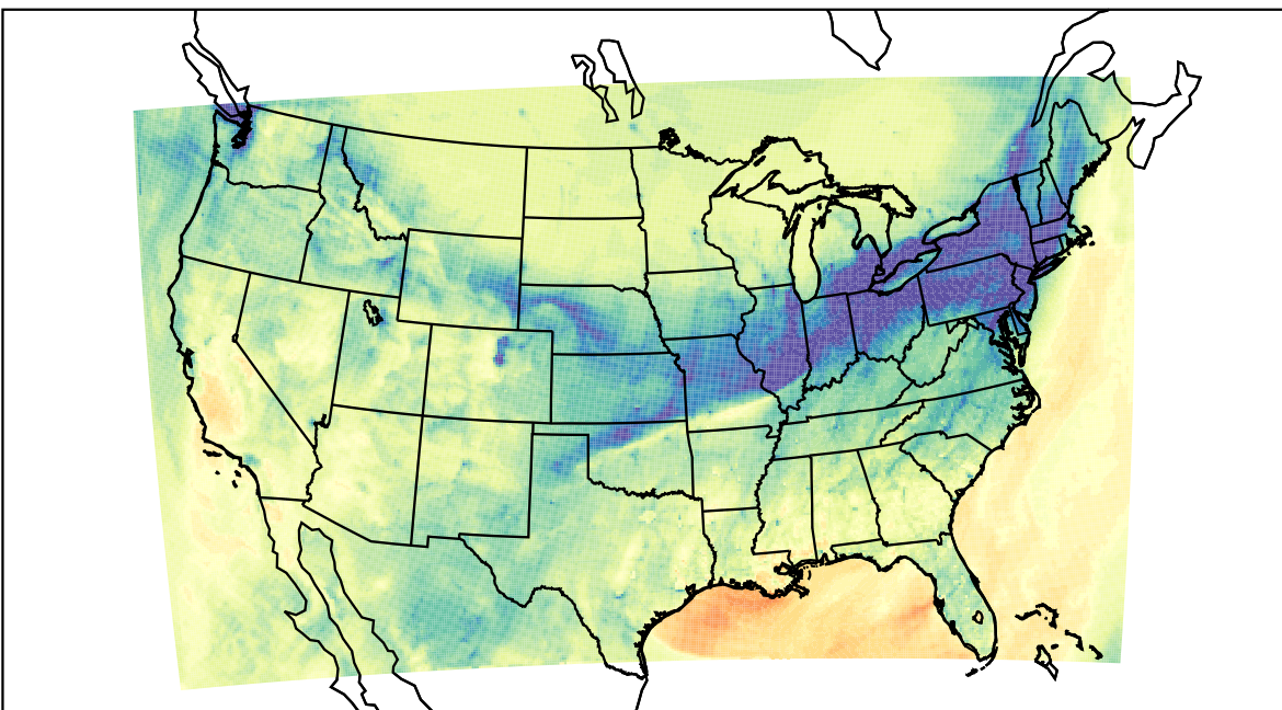
WRF (2019-11-10_23:00:00)
