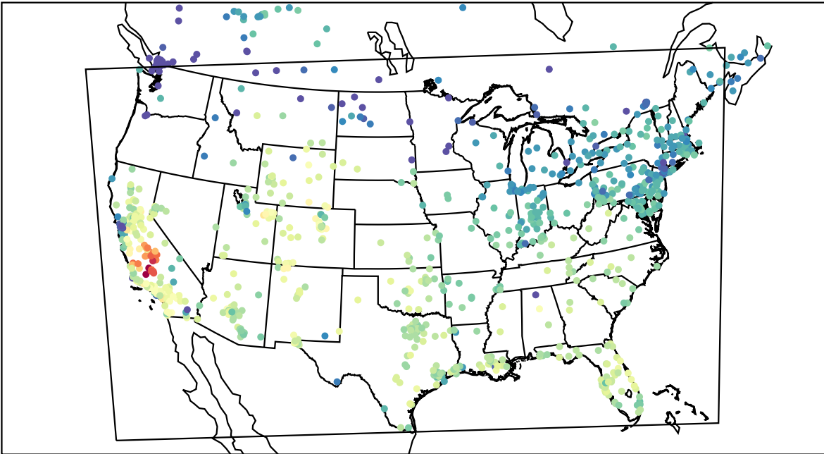
AirNOW (2019-11-09_20:00:00)
