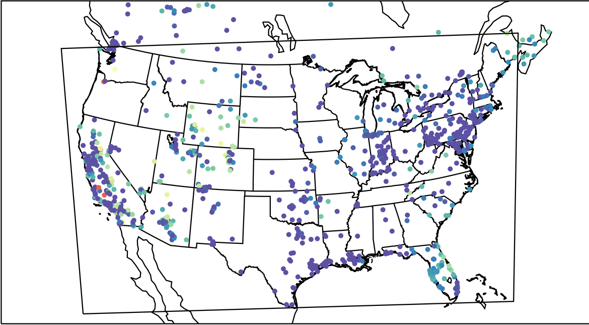
AirNOW (2019-11-09_08:00:00)
