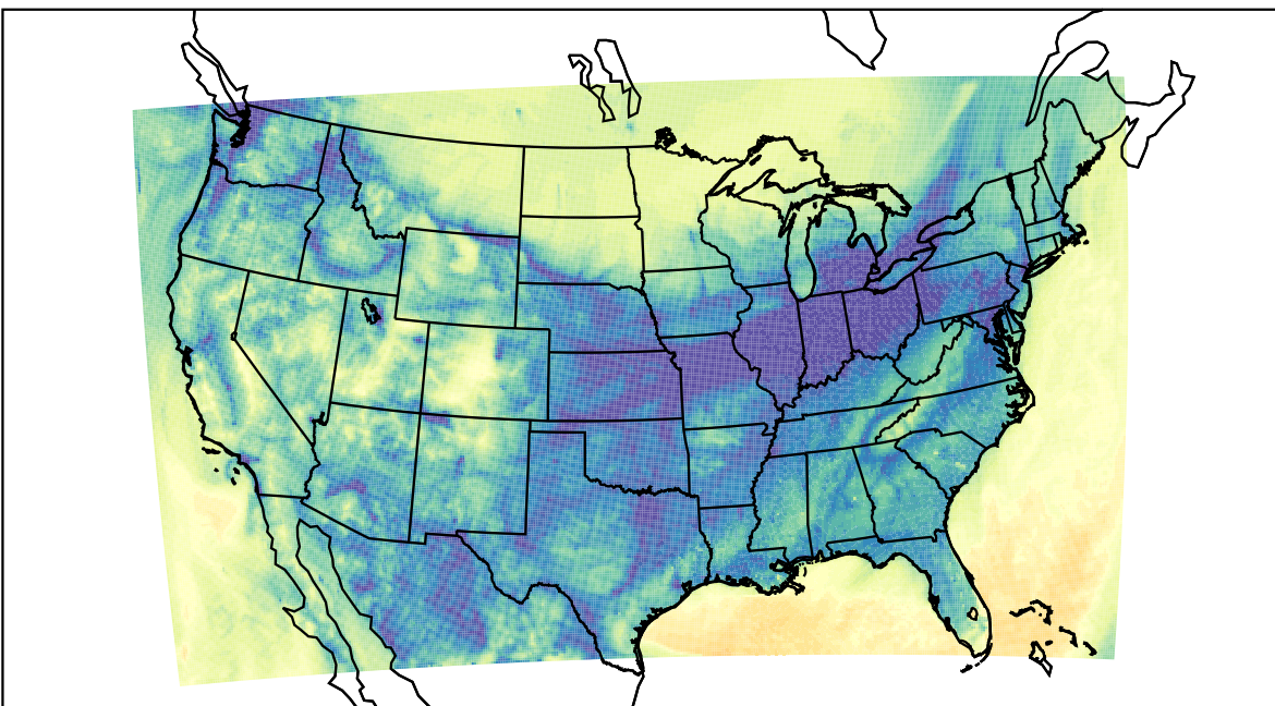
WRF (2019-11-10_14:00:00)
