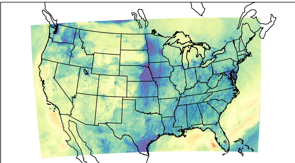
WRF (2019-11-09_00:00:00)
