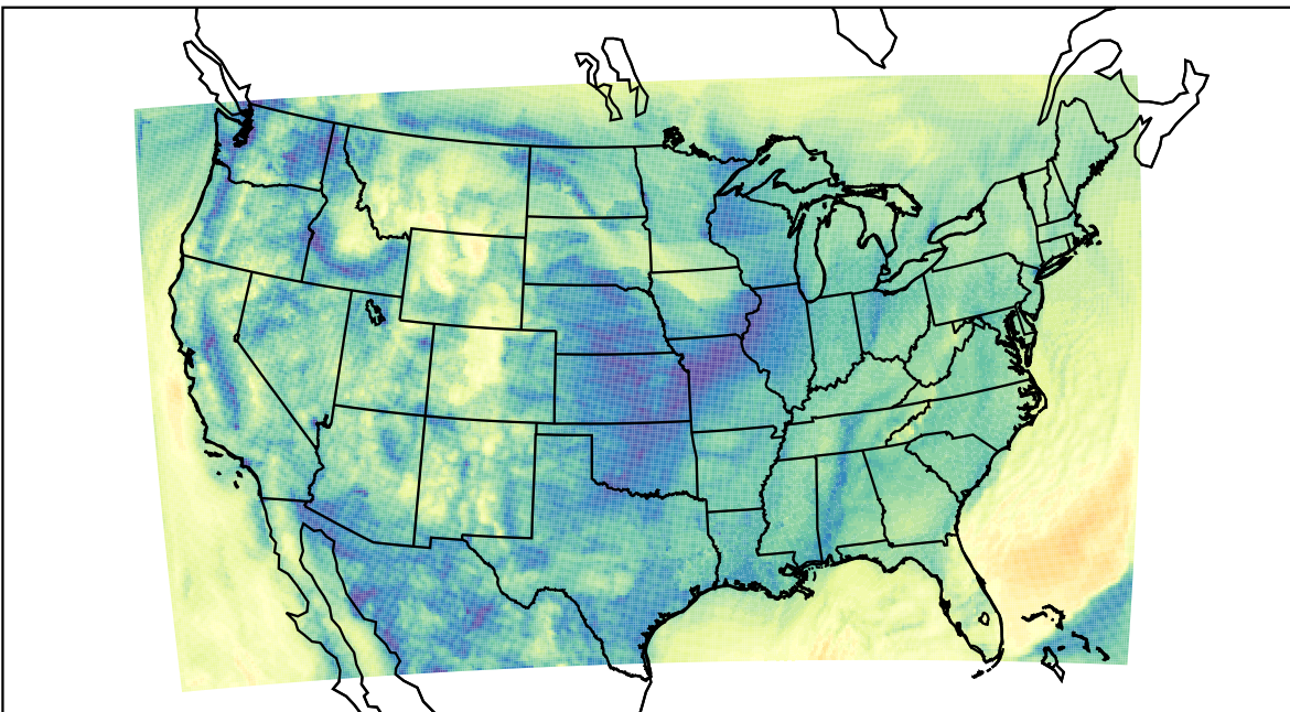
WRF (2019-11-09_16:00:00)
