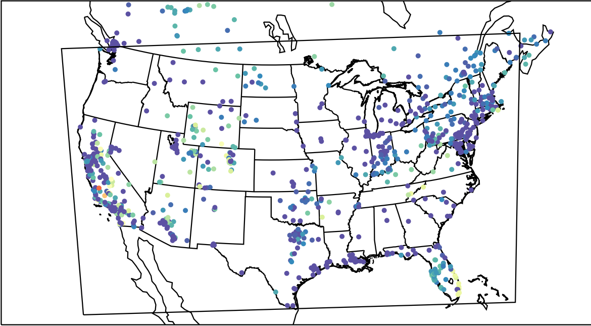
AirNOW (2019-11-10_08:00:00)
