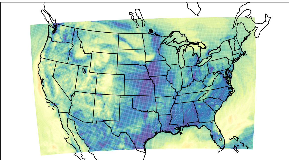
WRF (2019-11-09_08:00:00)
