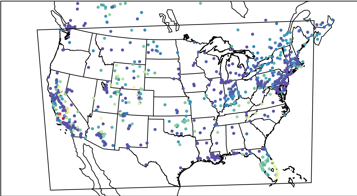
AirNOW (2019-11-10_04:00:00)
