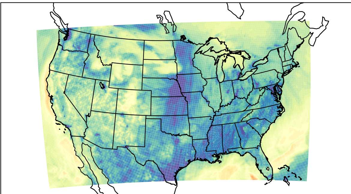
WRF (2019-11-09_04:00:00)
