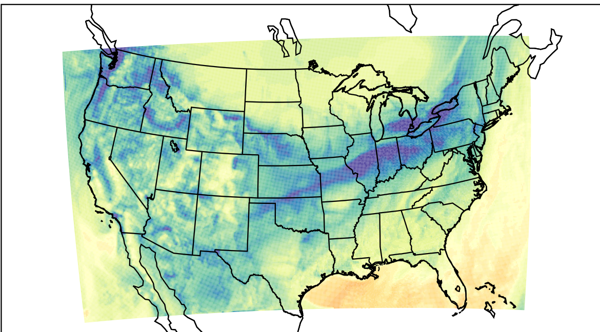
WRF (2019-11-10_17:00:00)
