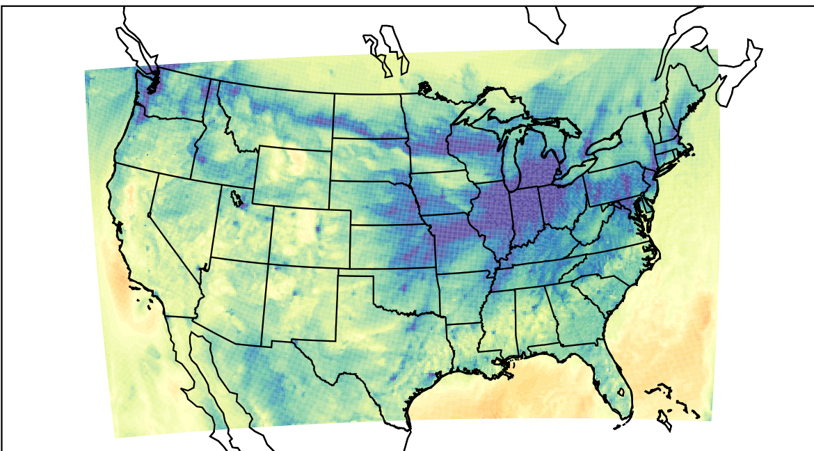
WRF (2019-11-10_00:00:00)
