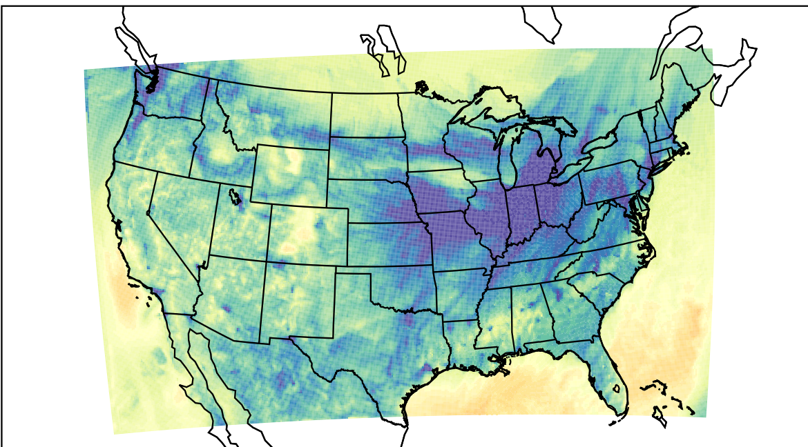
WRF (2019-11-10_04:00:00)
