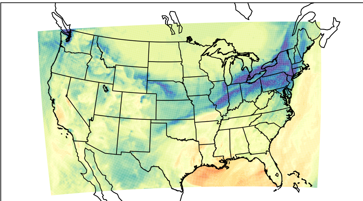
WRF (2019-11-10_21:00:00)
