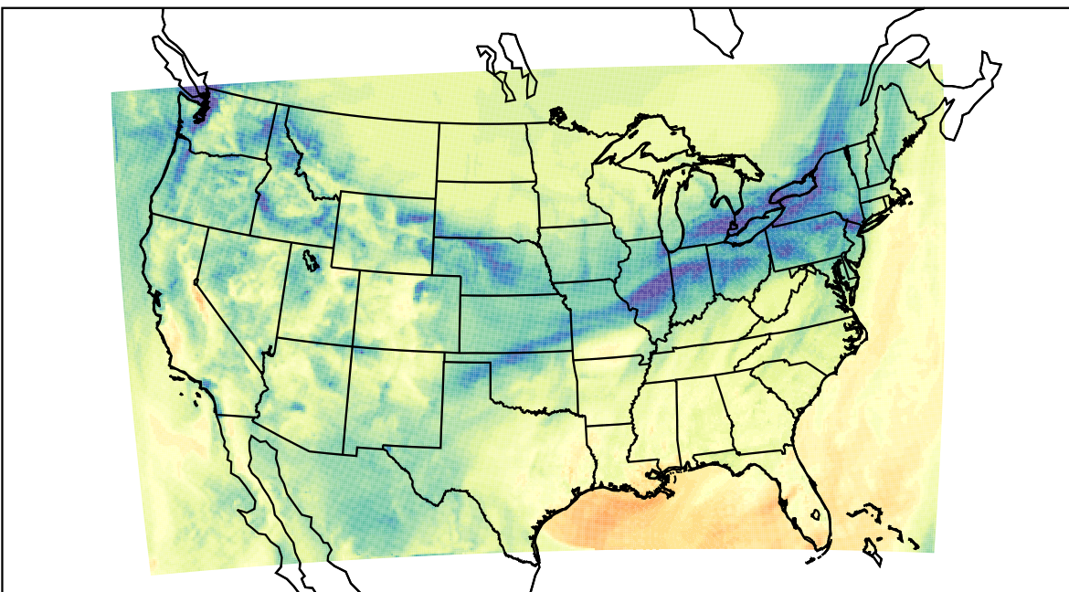
WRF (2019-11-10_19:00:00)
