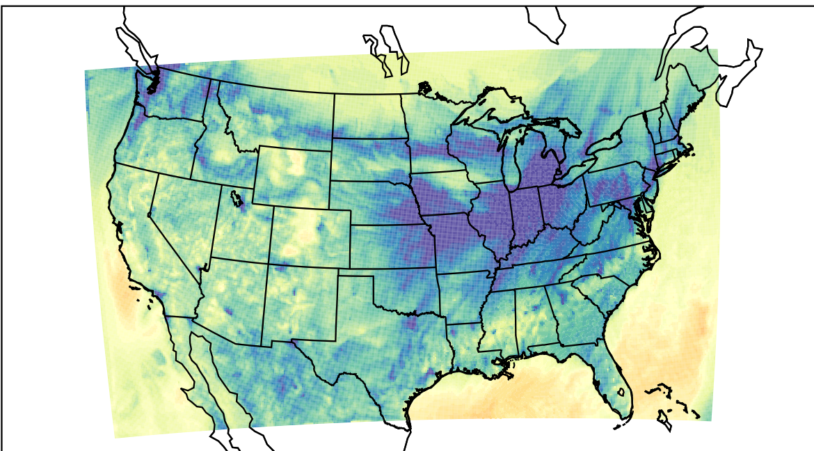
WRF (2019-11-10_03:00:00)
