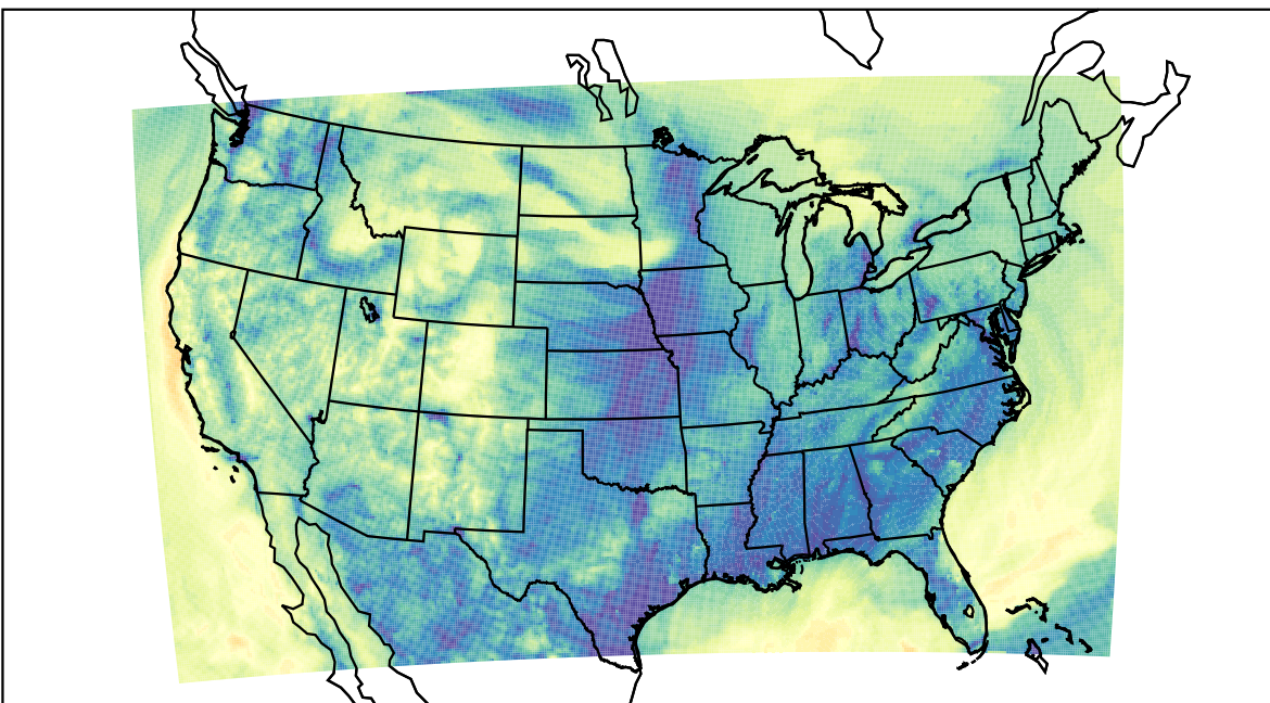
WRF (2019-11-09_07:00:00)
