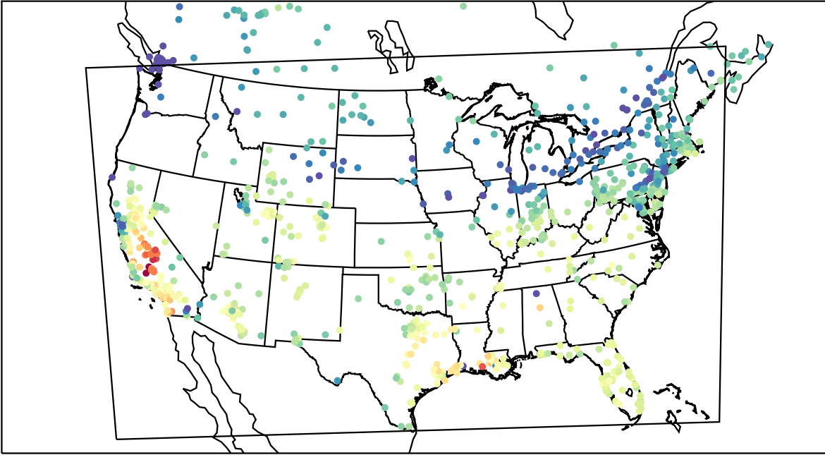
AirNOW (2019-11-10_20:00:00)
