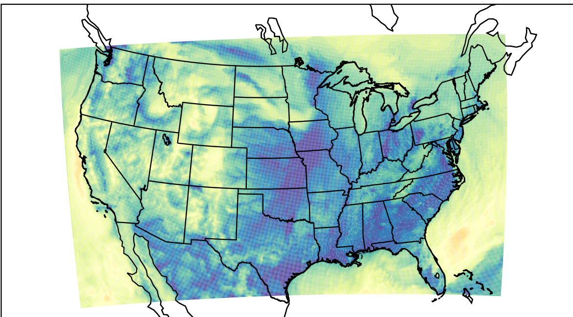
WRF (2019-11-09_11:00:00)
