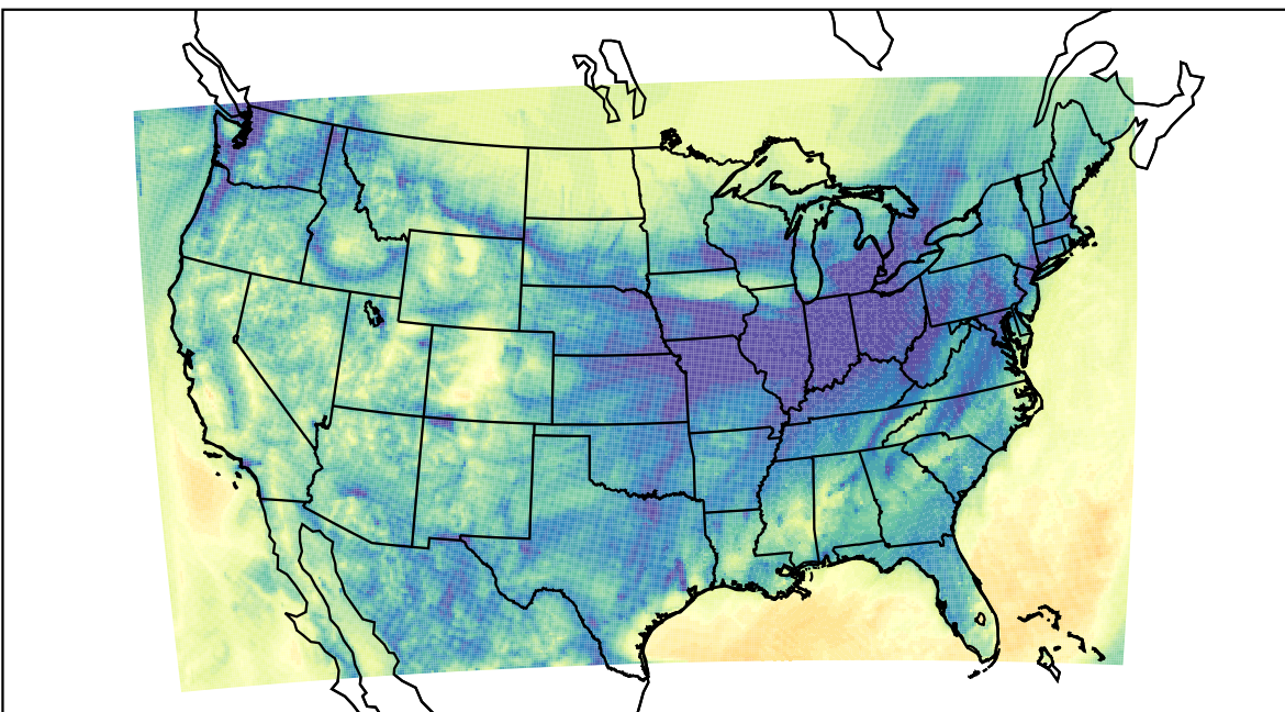
WRF (2019-11-10_08:00:00)
