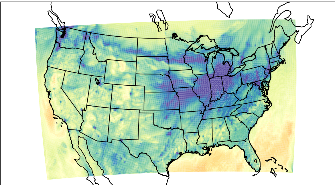
WRF (2019-11-10_01:00:00)
