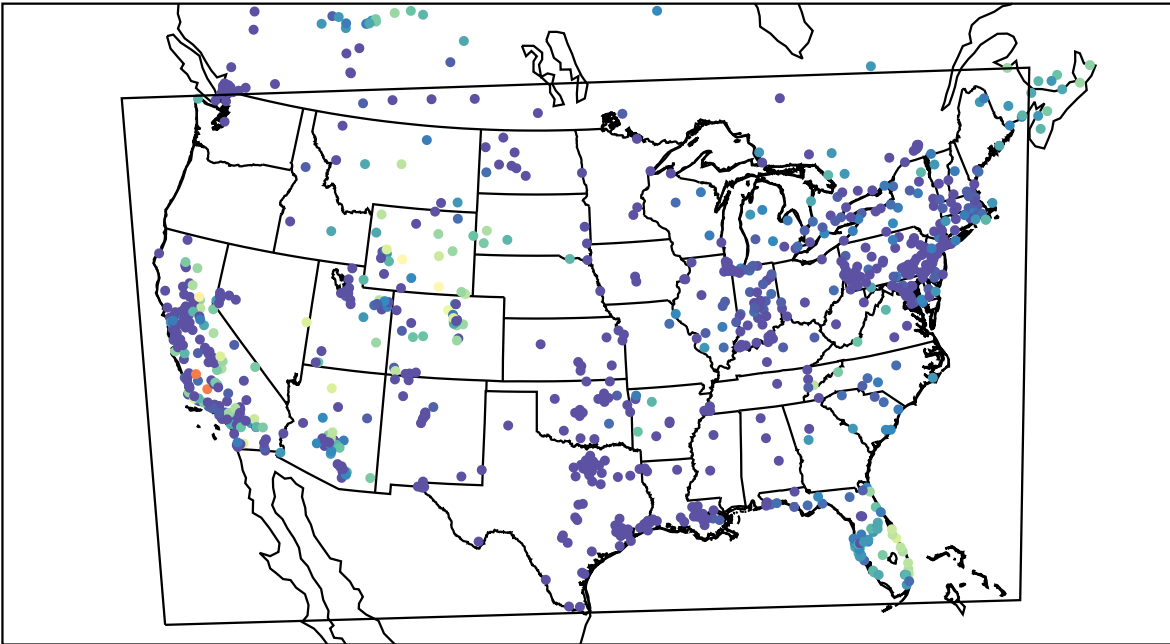
AirNOW (2019-11-09_13:00:00)
