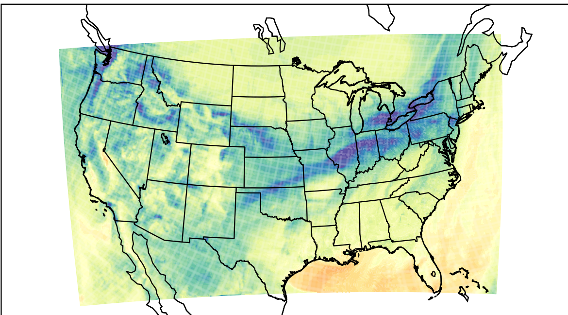
WRF (2019-11-10_18:00:00)
