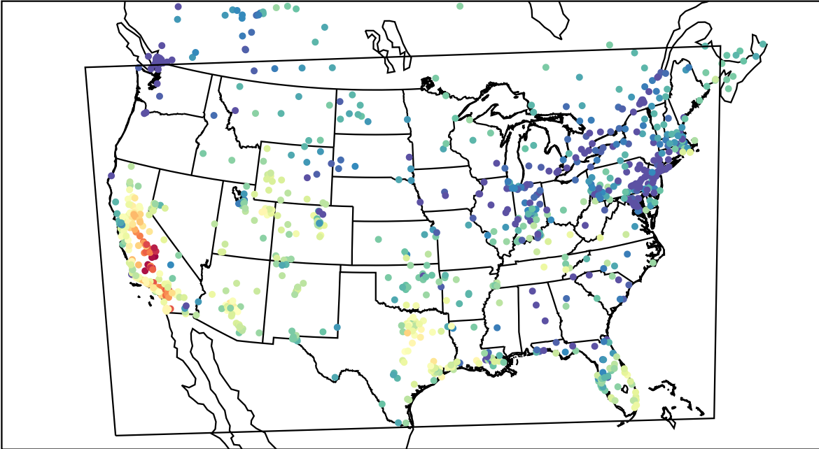
AirNOW (2019-11-10_23:00:00)
