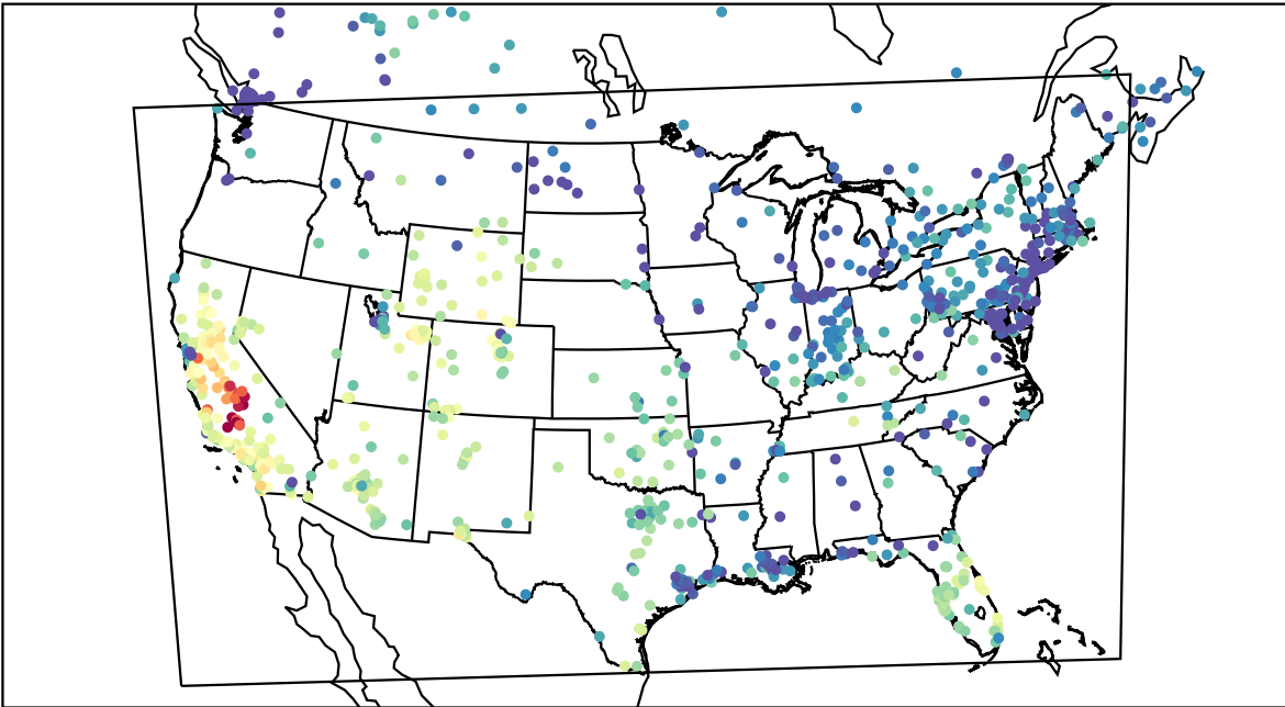
AirNOW (2019-11-09_23:00:00)
