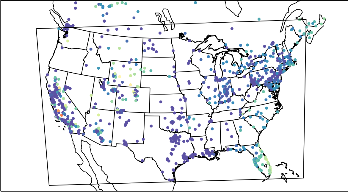
AirNOW (2019-11-09_14:00:00)
