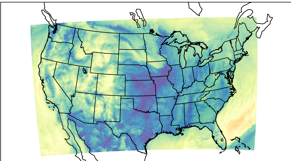
WRF (2019-11-09_14:00:00)
