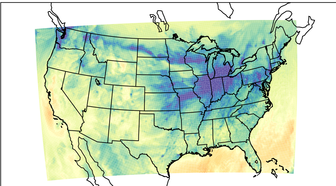
WRF (2019-11-09_23:00:00)
