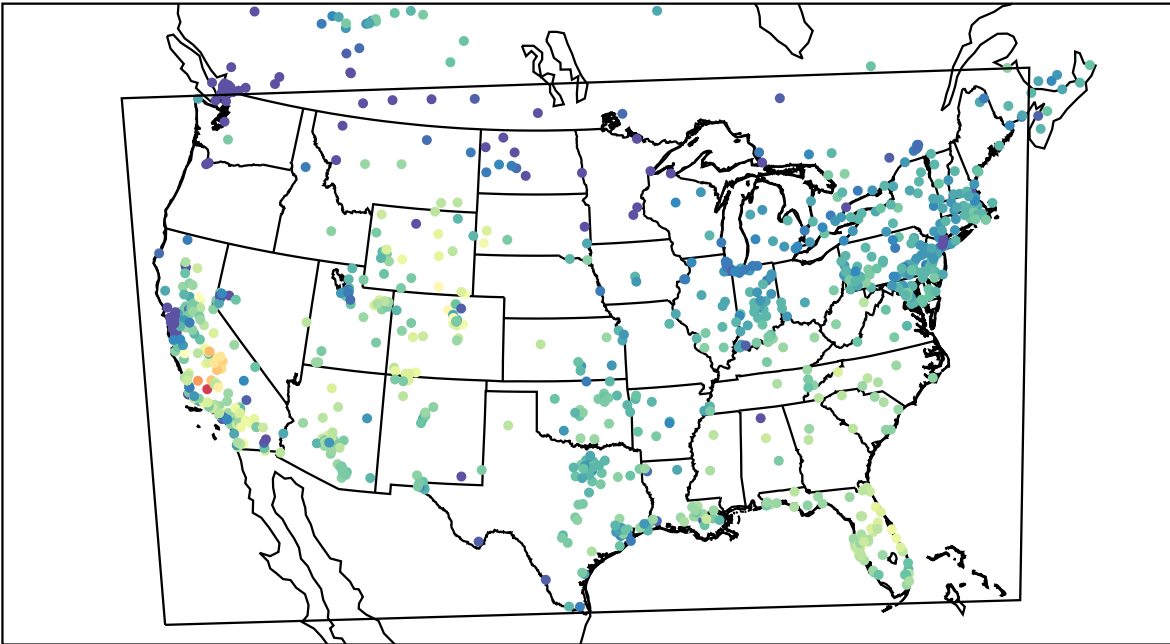
AirNOW (2019-11-09_18:00:00)
