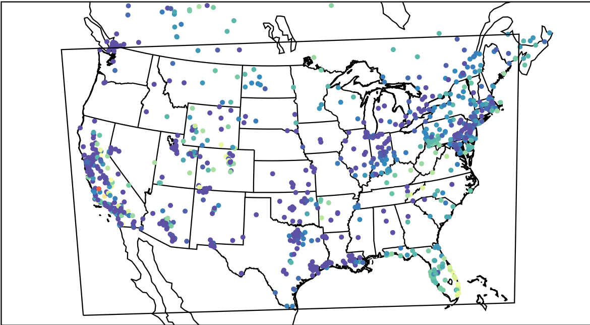
AirNOW (2019-11-10_14:00:00)
