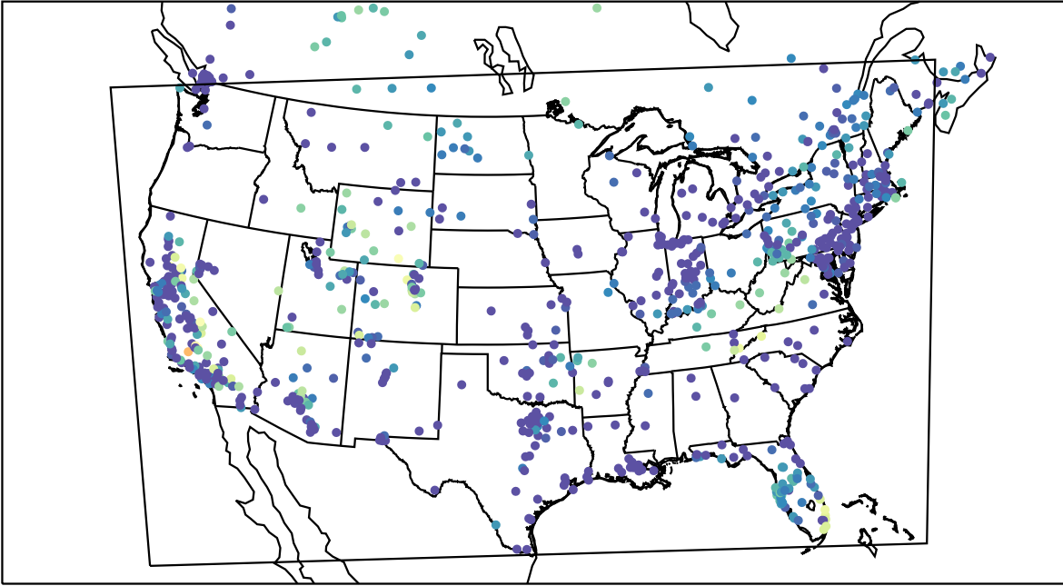
AirNOW (2019-11-10_10:00:00)
