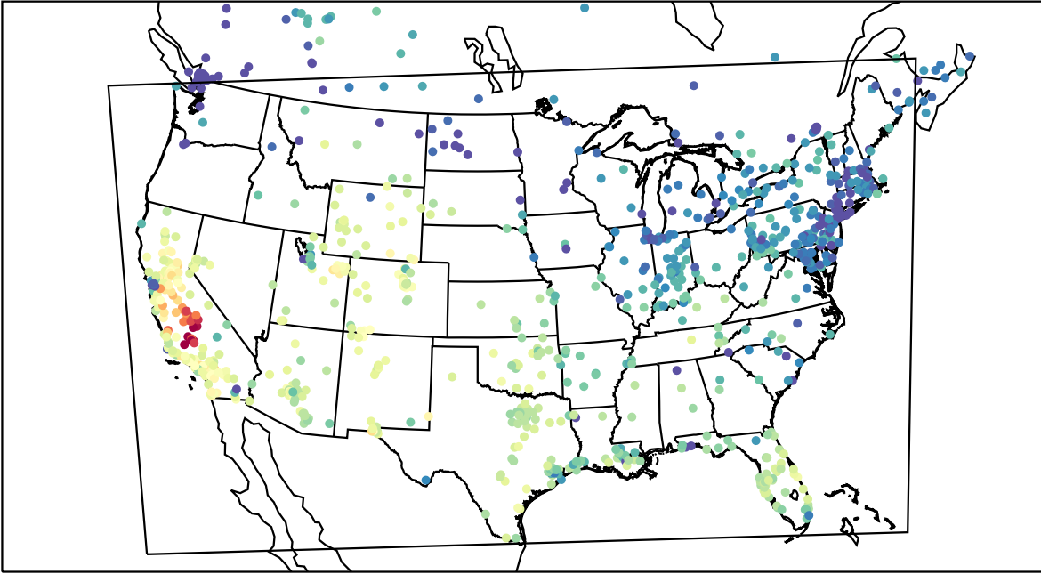
AirNOW (2019-11-09_22:00:00)
