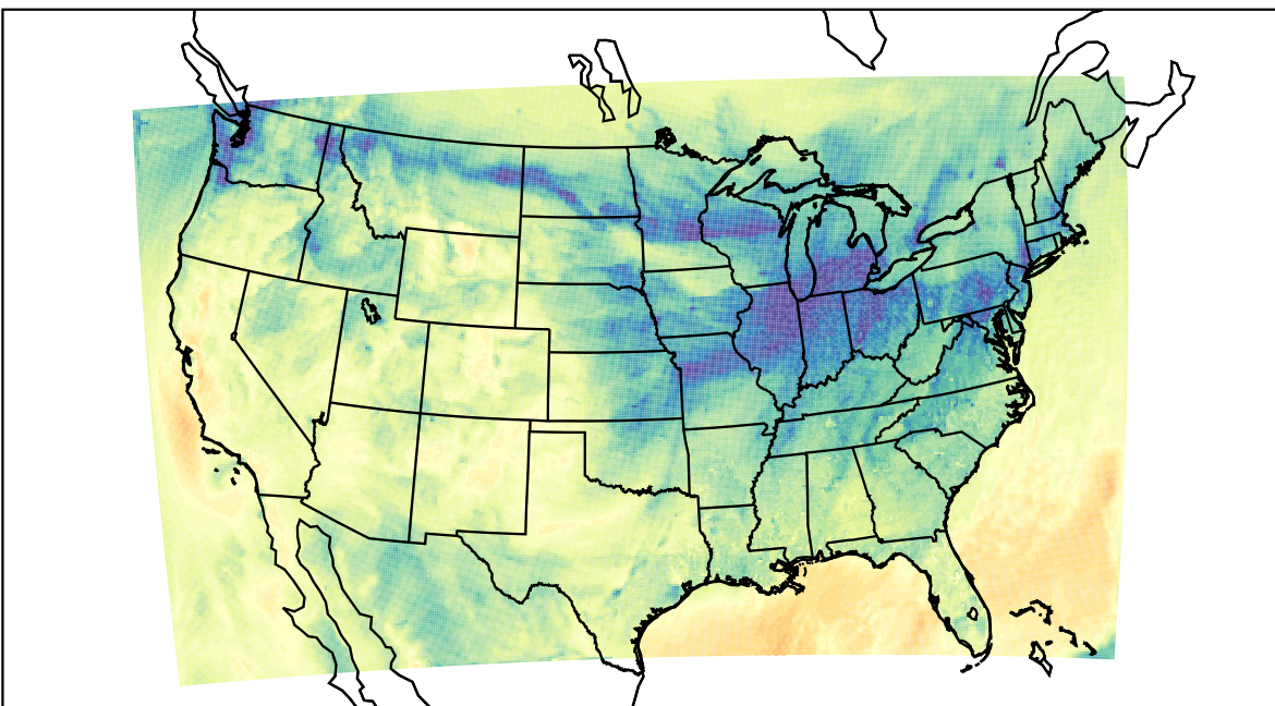
WRF (2019-11-09_22:00:00)
