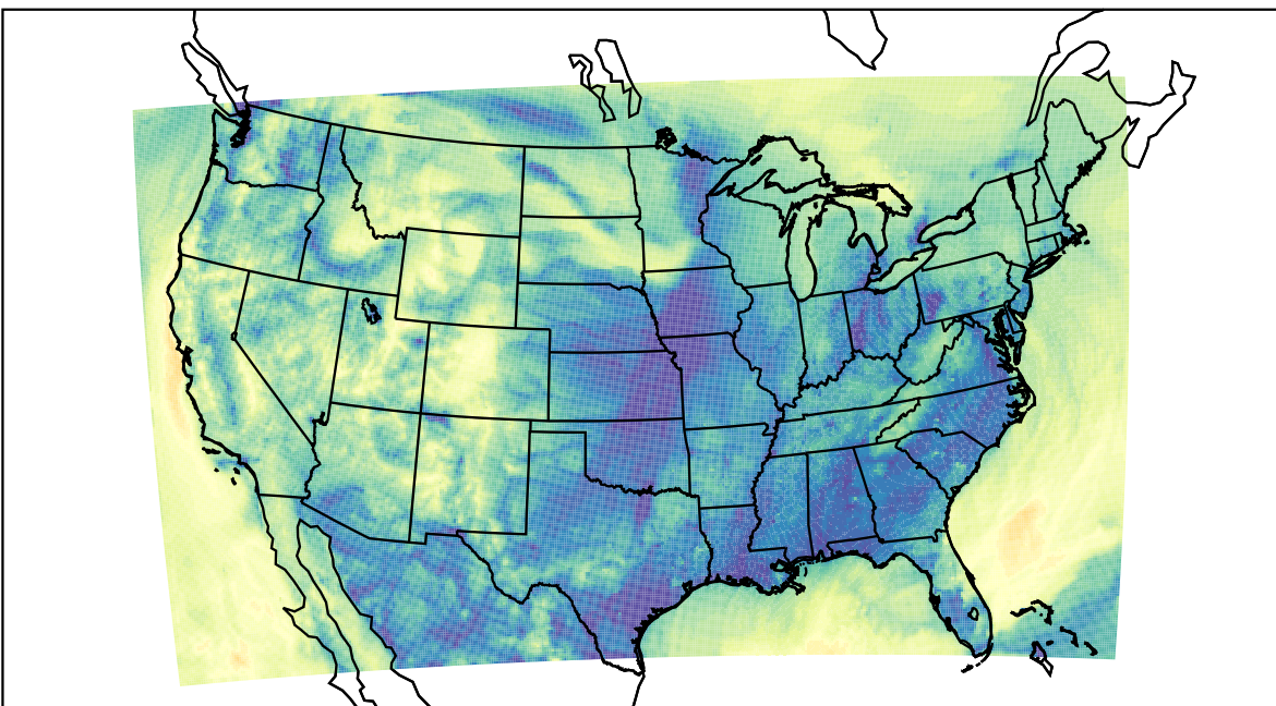
WRF (2019-11-09_10:00:00)
