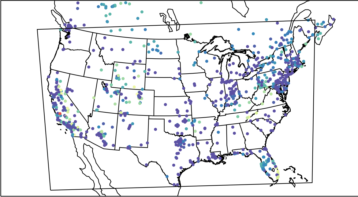
AirNOW (2019-11-10_11:00:00)
