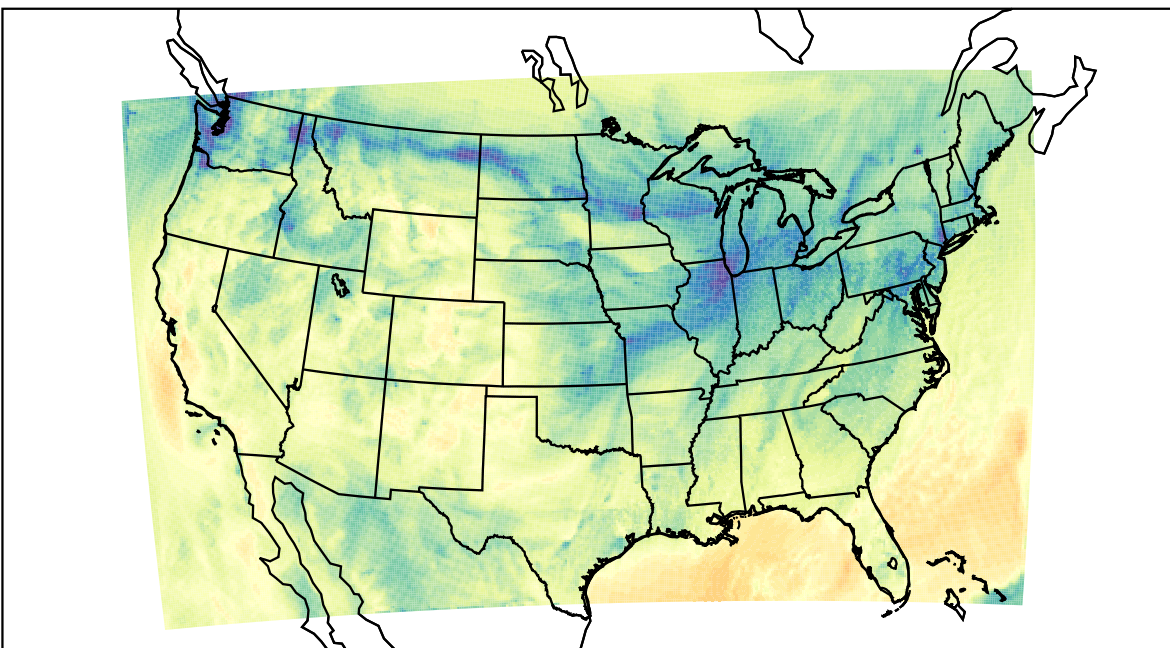
WRF (2019-11-09_21:00:00)
