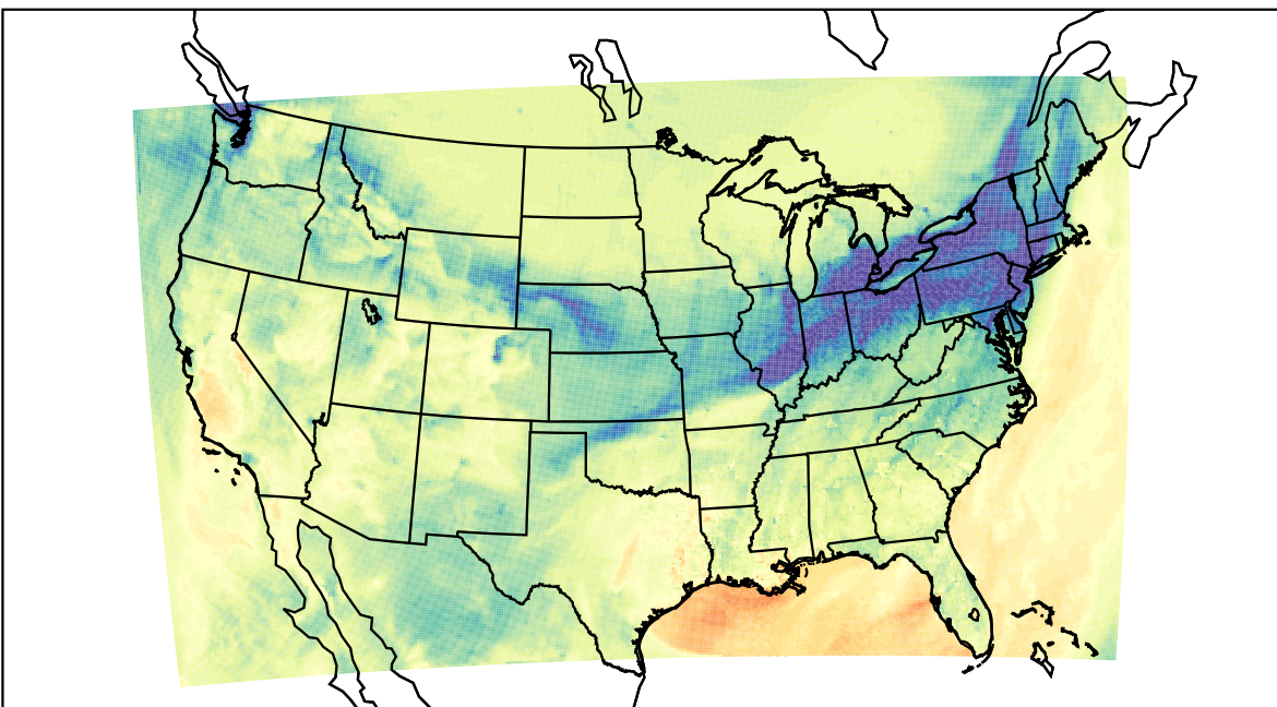
WRF (2019-11-10_22:00:00)
