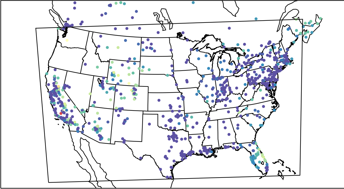
AirNOW (2019-11-09_10:00:00)
