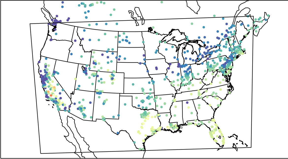
AirNOW (2019-11-10_17:00:00)
