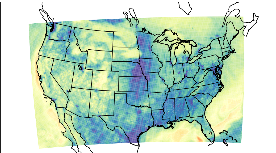
WRF (2019-11-09_03:00:00)
