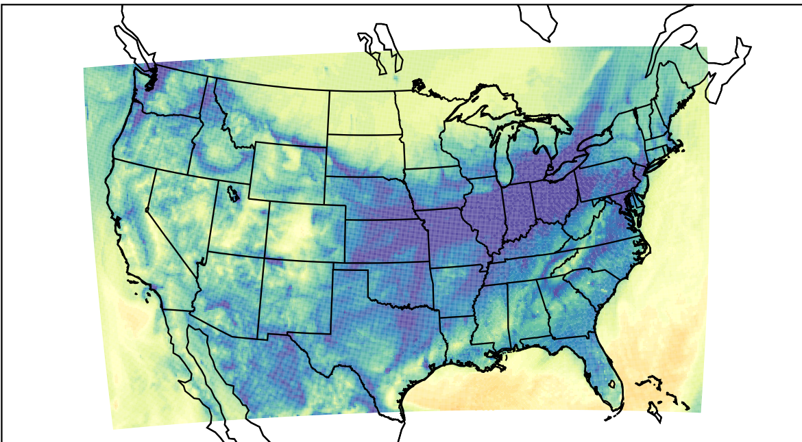
WRF (2019-11-10_13:00:00)
