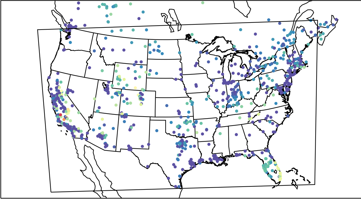
AirNOW (2019-11-10_06:00:00)
