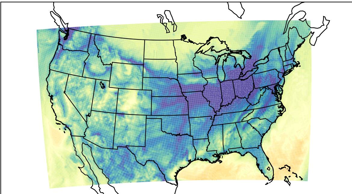
WRF (2019-11-10_10:00:00)
