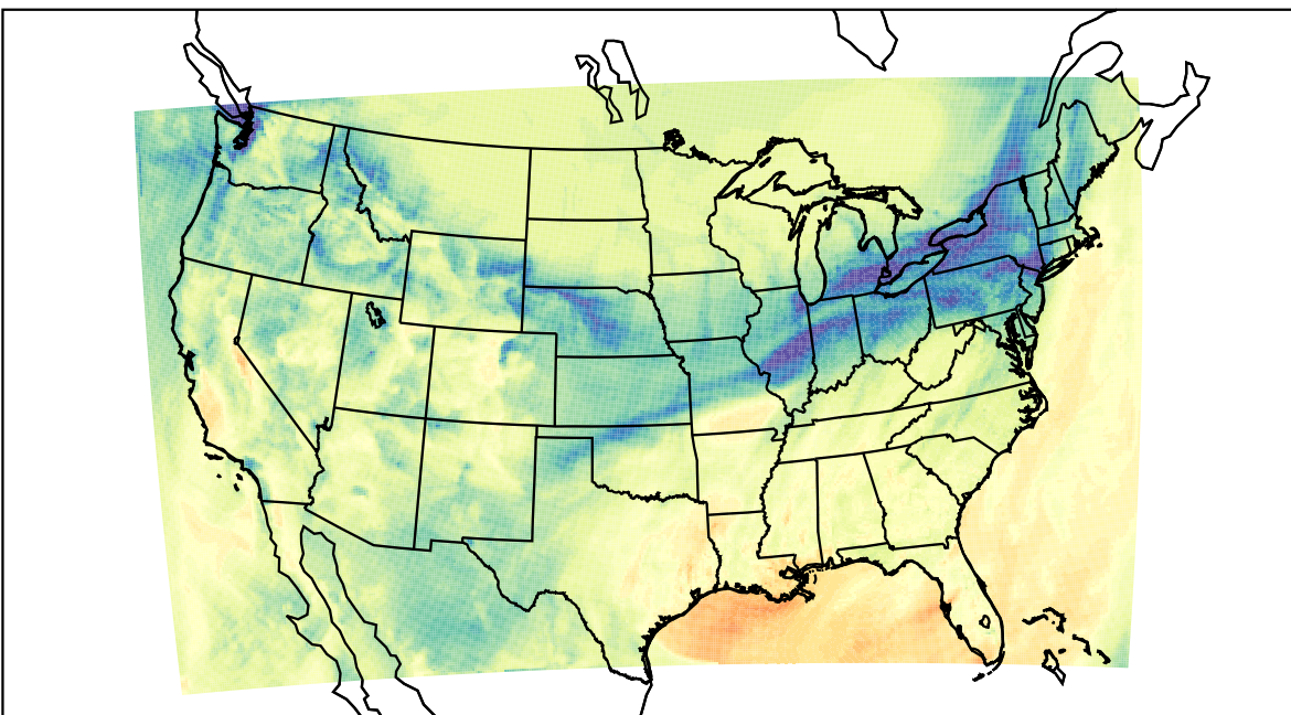
WRF (2019-11-10_20:00:00)
