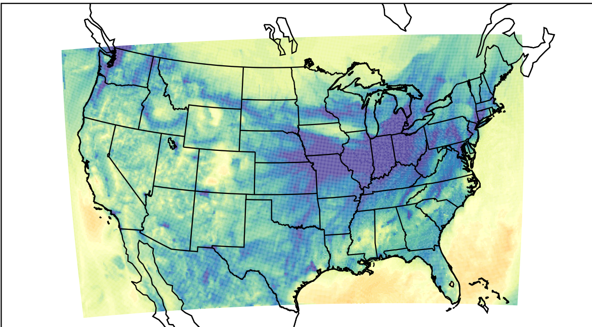
WRF (2019-11-10_06:00:00)
