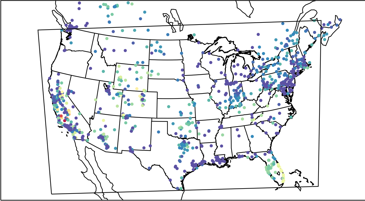
AirNOW (2019-11-10_03:00:00)
