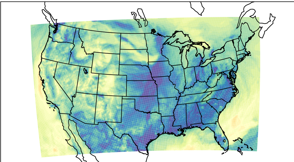
WRF (2019-11-09_09:00:00)
