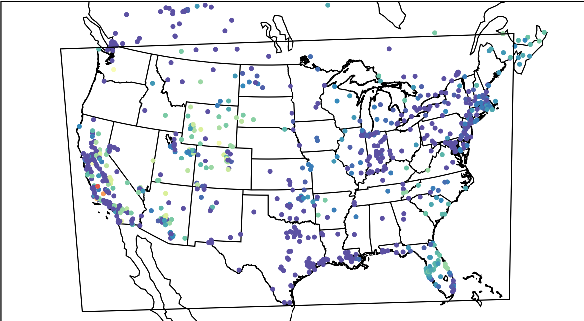
AirNOW (2019-11-09_06:00:00)
