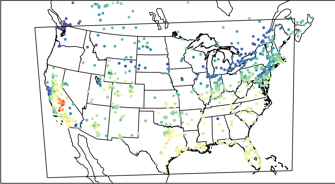
AirNOW (2019-11-10_19:00:00)
