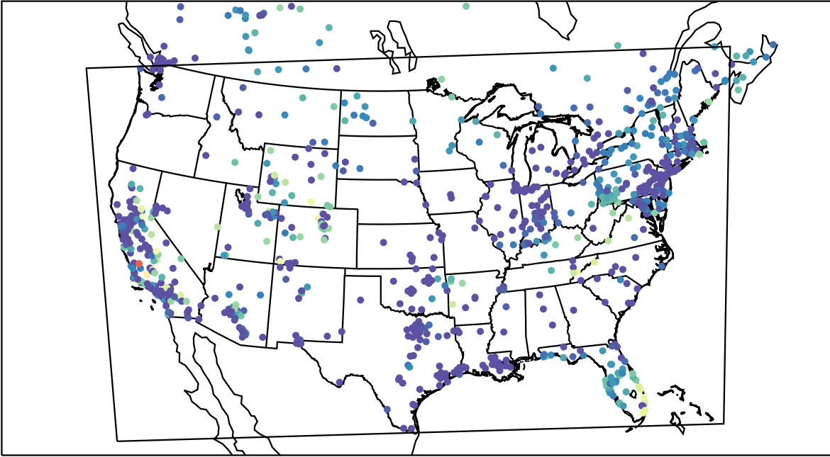
AirNOW (2019-11-10_13:00:00)
