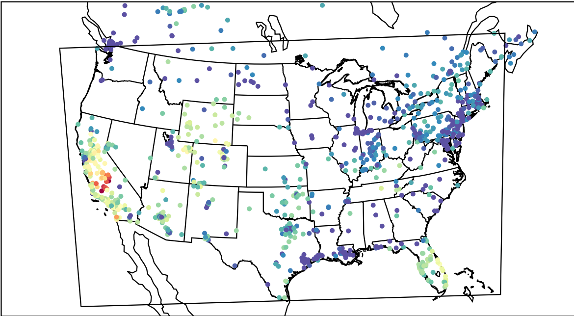
AirNOW (2019-11-10_00:00:00)
