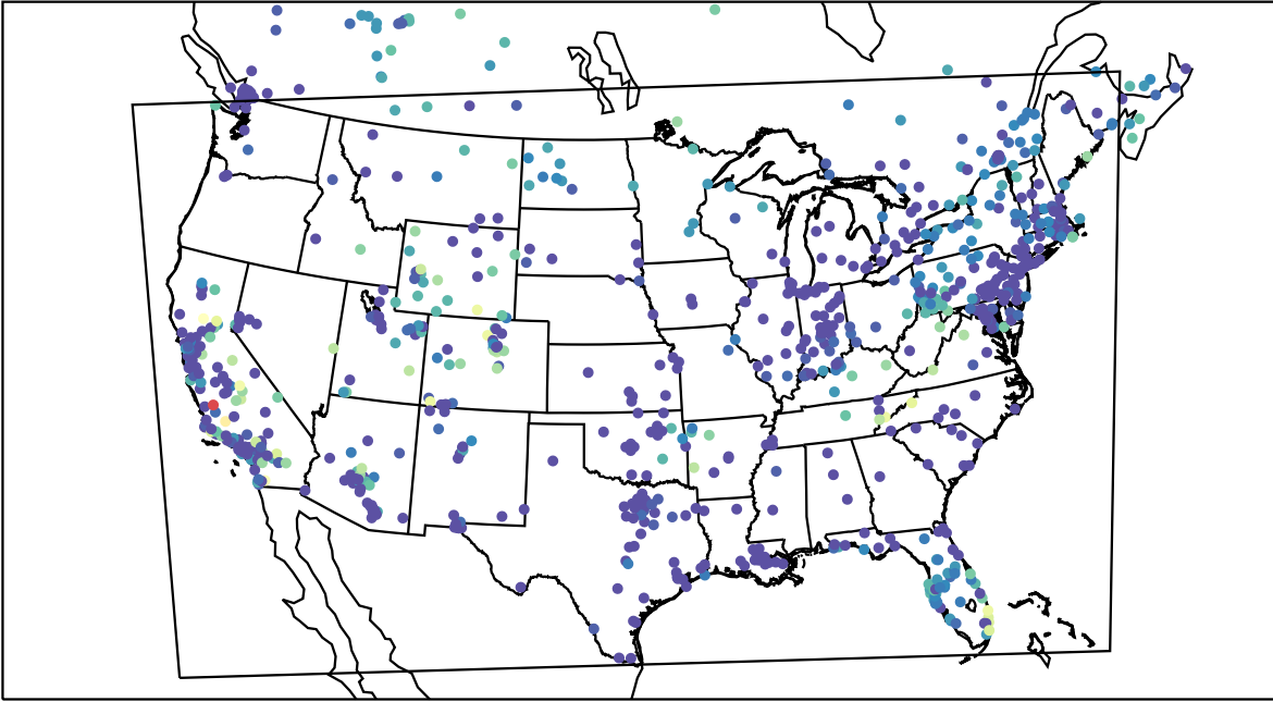
AirNOW (2019-11-10_12:00:00)
