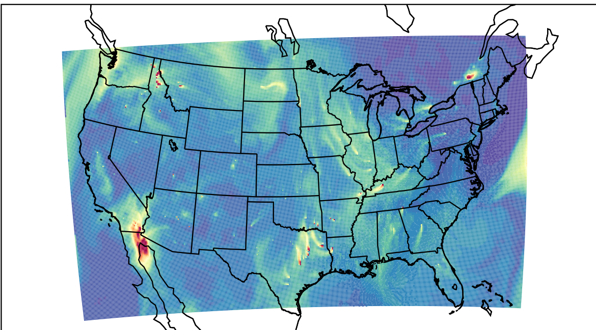
WRF 2019-11-16_20:00:00
