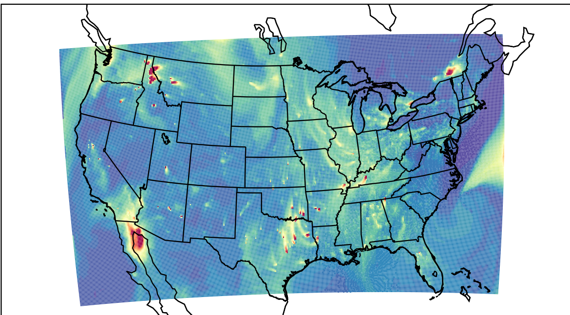
WRF 2019-11-16_23:00:00
