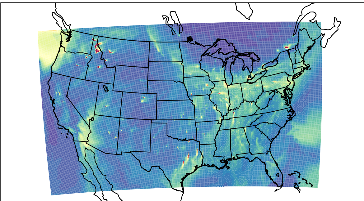
WRF 2019-11-15_22:00:00
