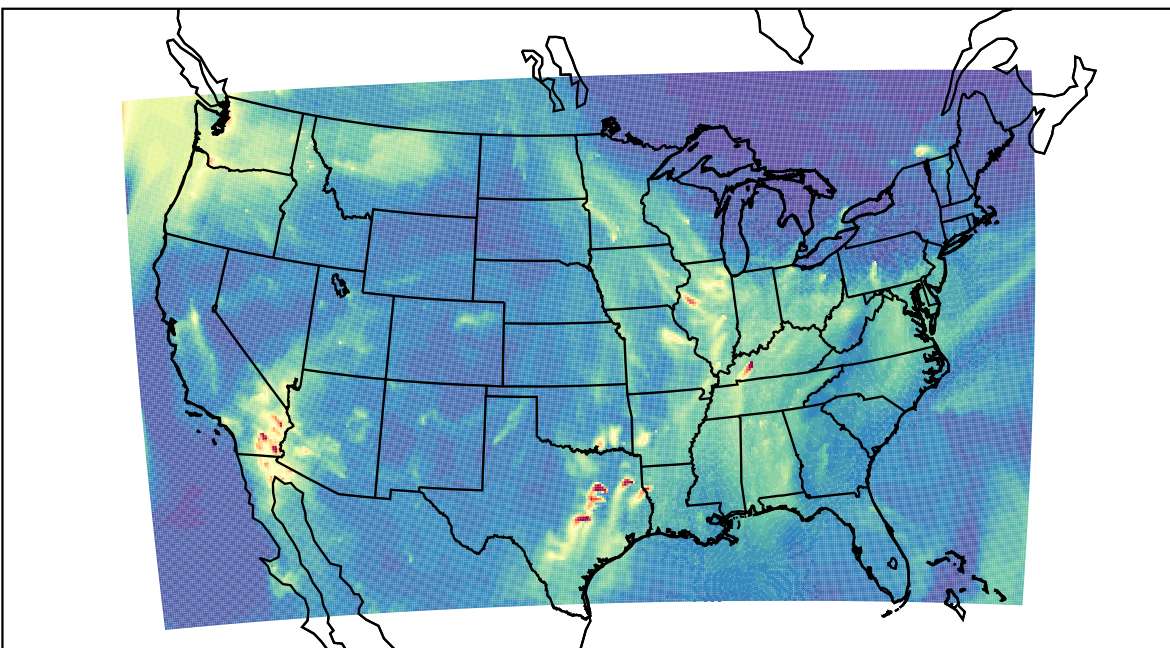
WRF 2019-11-16_08:00:00
