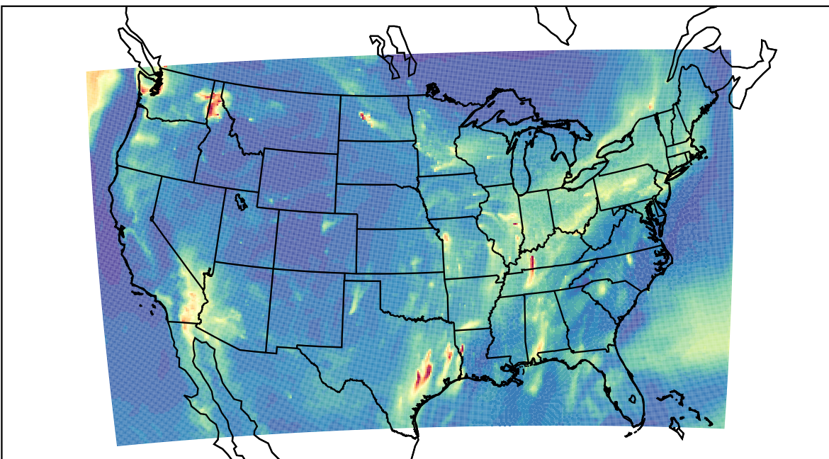
WRF 2019-11-15_09:00:00
