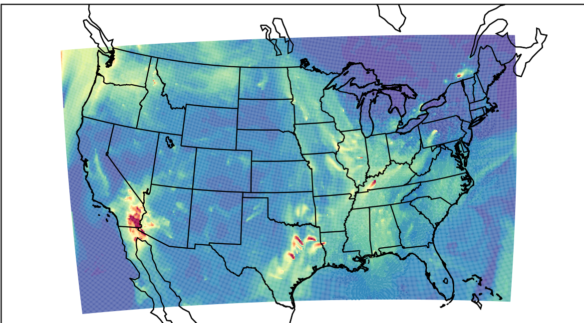
WRF 2019-11-16_12:00:00
