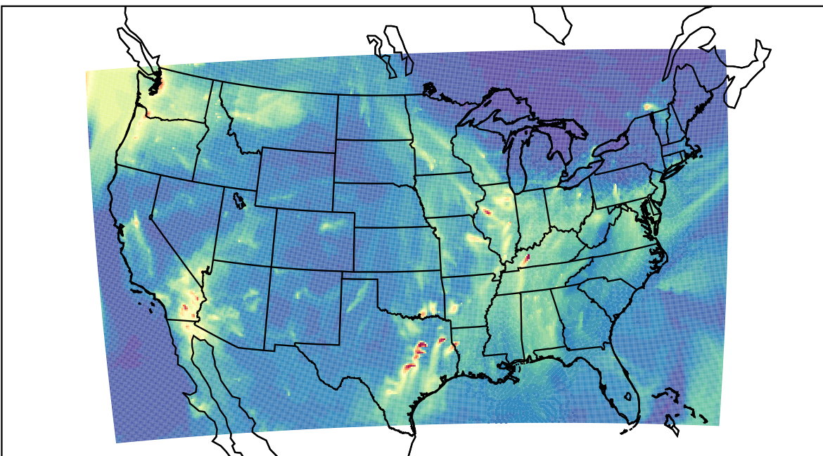
WRF 2019-11-16_07:00:00
