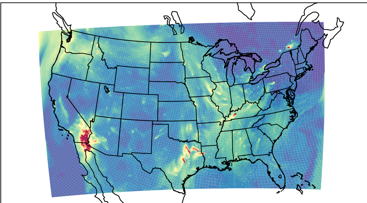
WRF 2019-11-16_14:00:00
