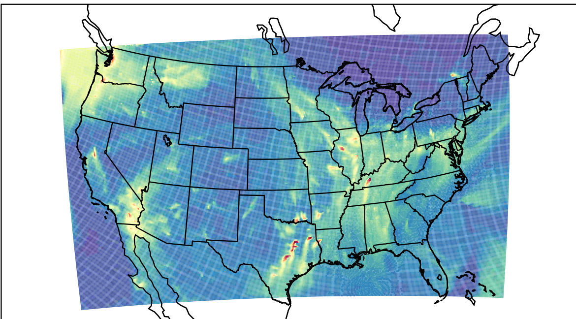
WRF 2019-11-16_06:00:00
