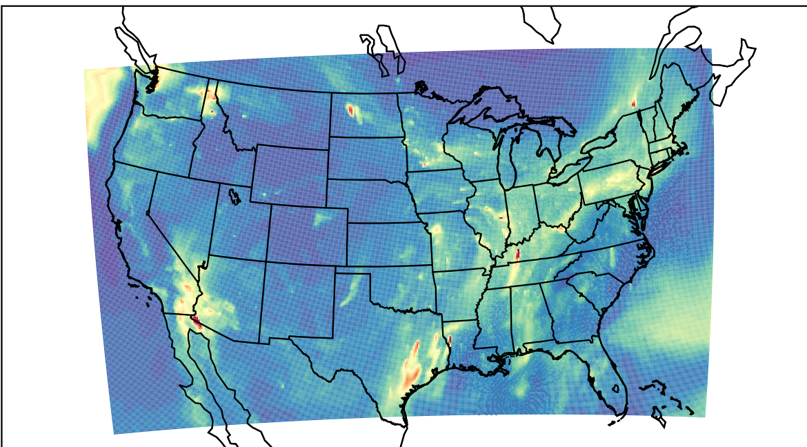
WRF 2019-11-15_12:00:00
