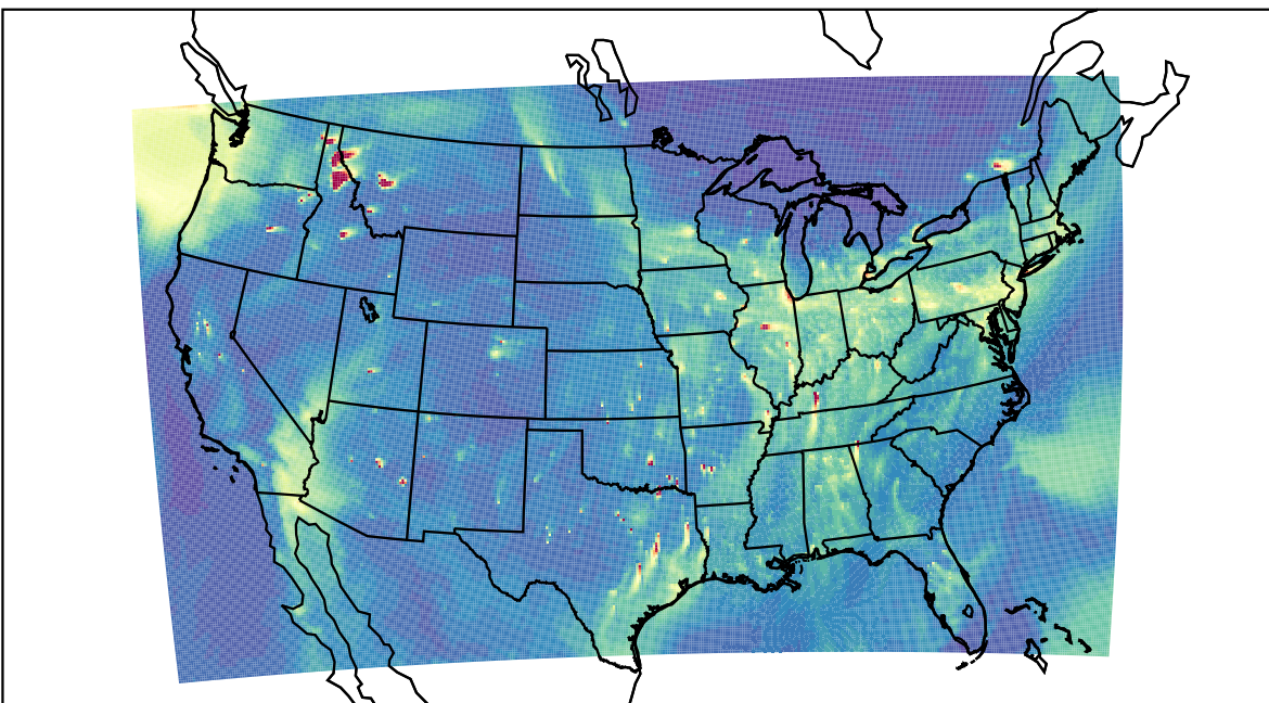
WRF 2019-11-15_23:00:00
