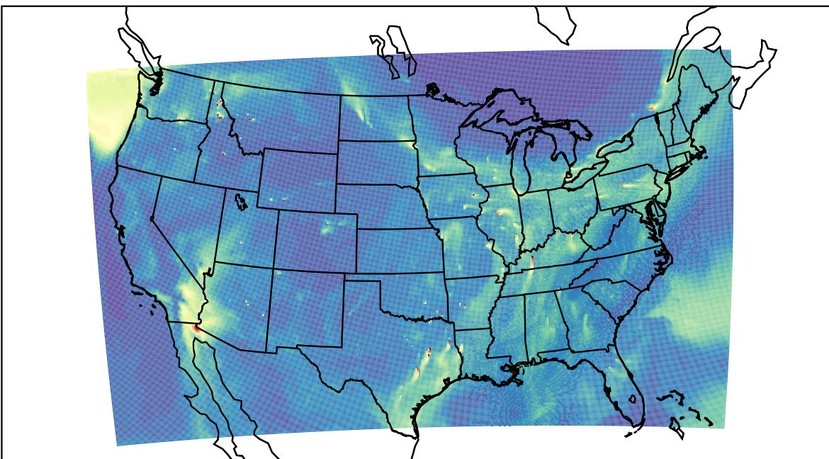
WRF 2019-11-15_19:00:00
