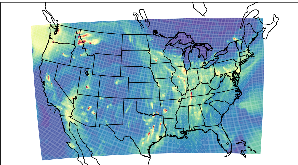
WRF 2019-11-16_03:00:00
