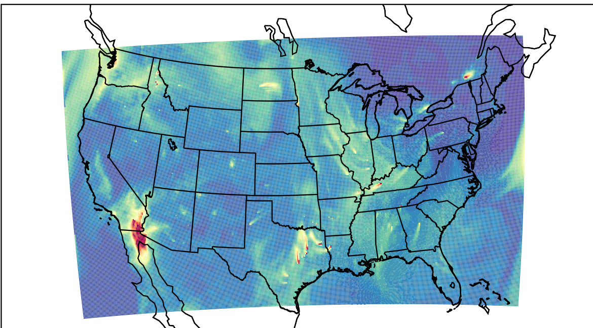
WRF 2019-11-16_18:00:00
