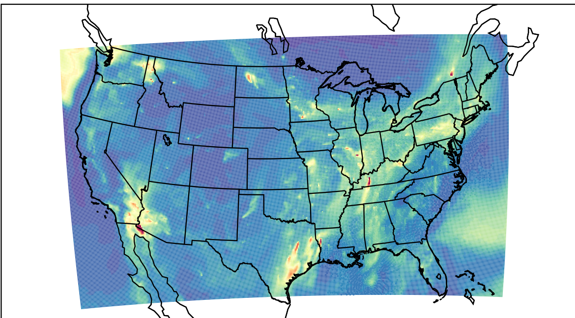
WRF 2019-11-15_13:00:00
