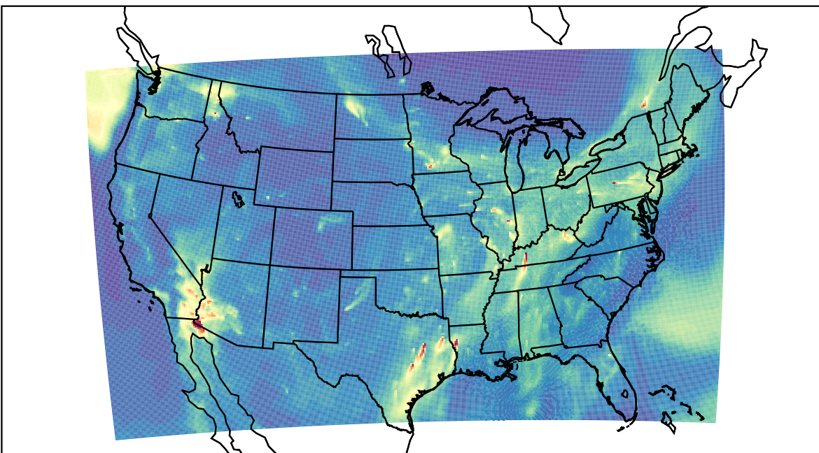
WRF 2019-11-15_15:00:00
