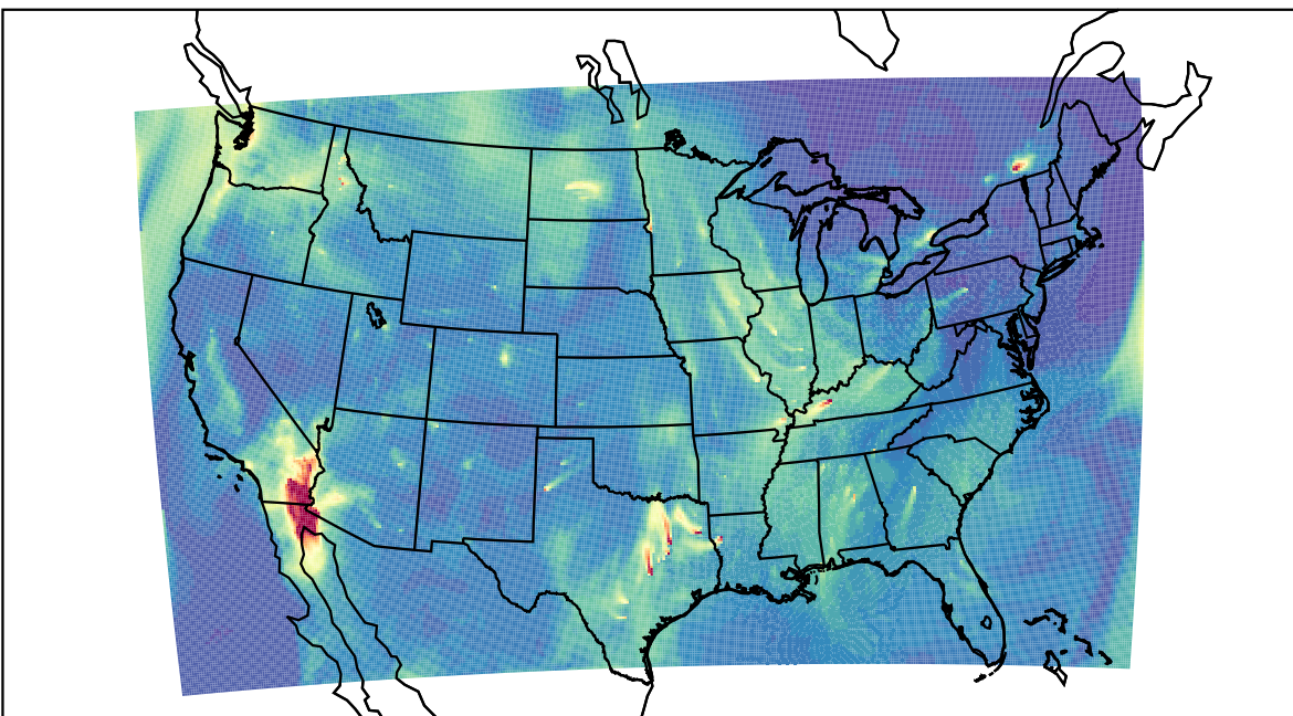
WRF 2019-11-16_17:00:00
