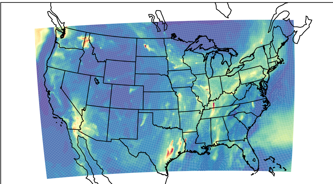
WRF 2019-11-15_10:00:00
