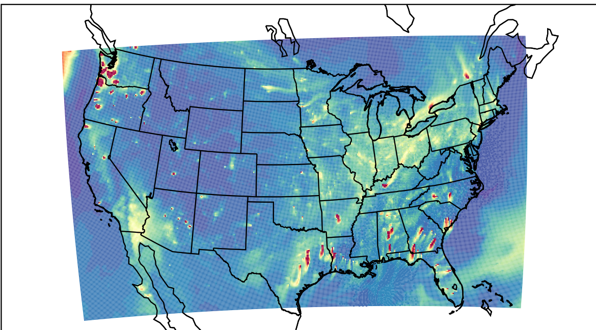
WRF 2019-11-15_00:00:00
