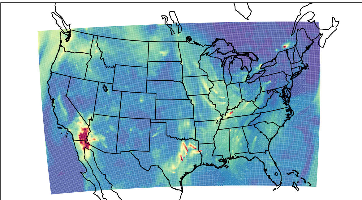
WRF 2019-11-16_15:00:00
