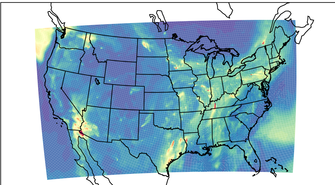
WRF 2019-11-15_14:00:00
