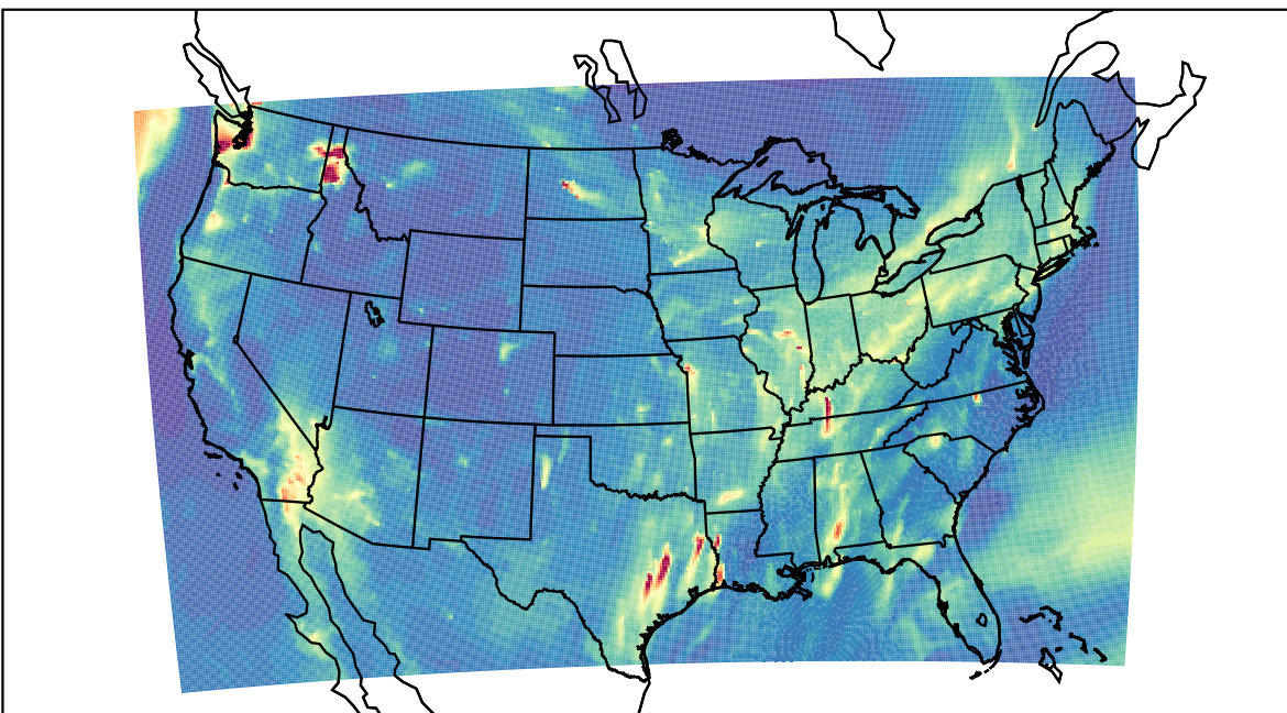
WRF 2019-11-15_07:00:00
