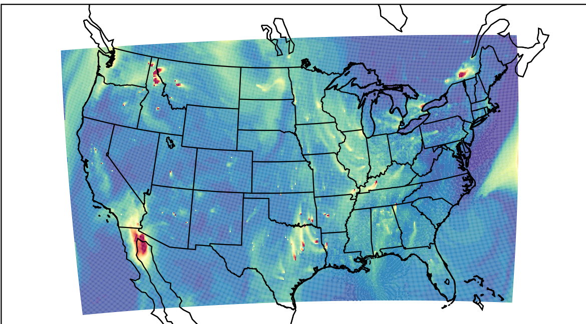
WRF 2019-11-16_22:00:00
