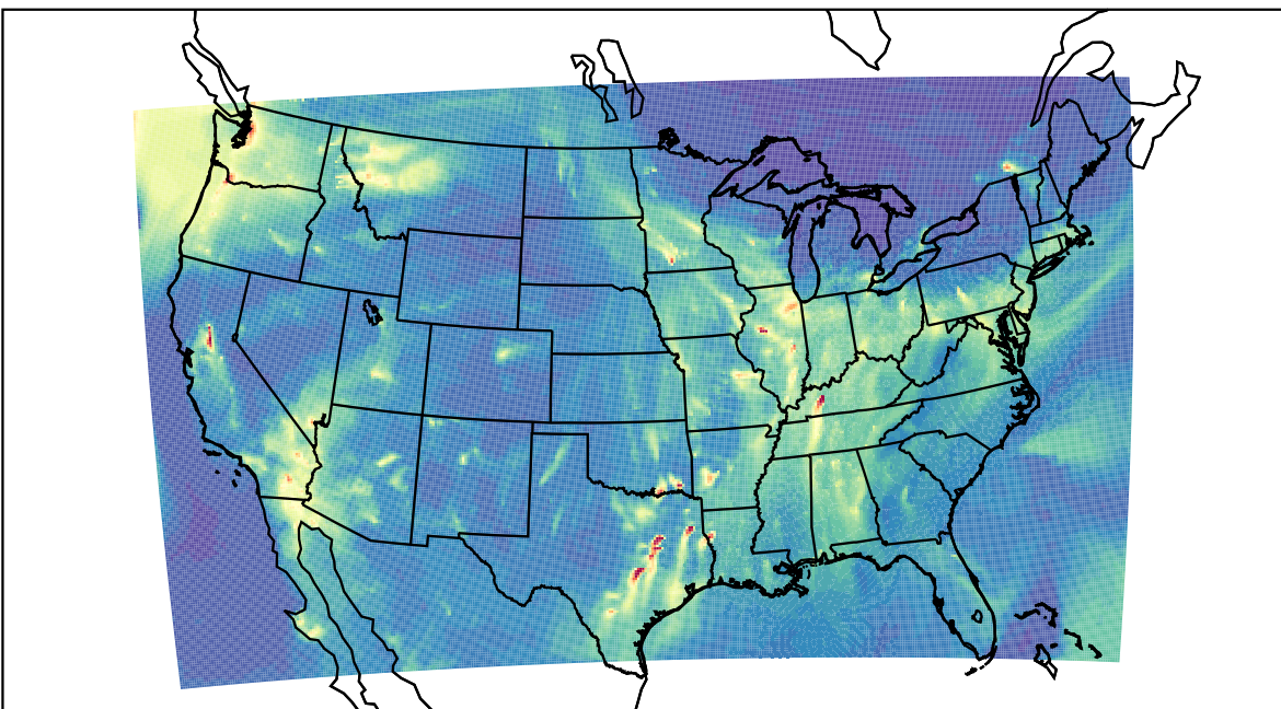
WRF 2019-11-16_05:00:00
