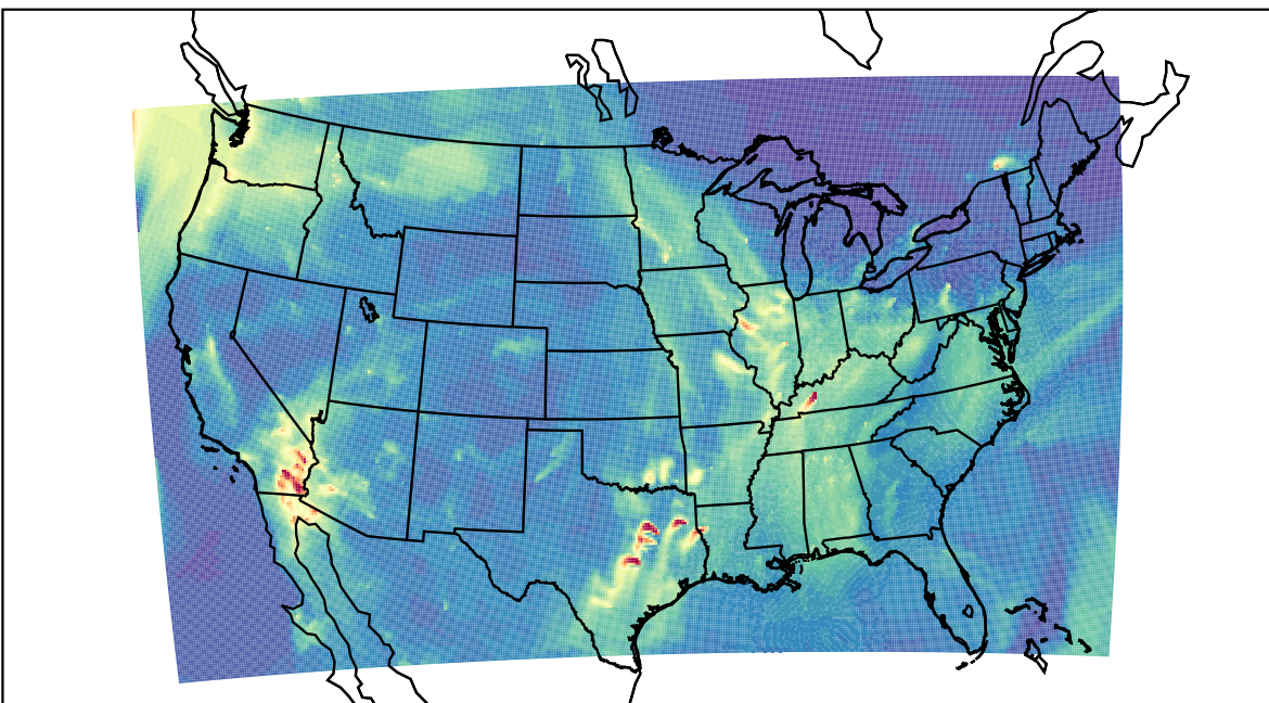
WRF 2019-11-16_09:00:00
