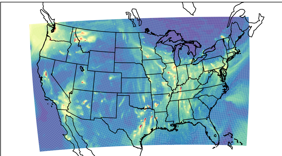
WRF 2019-11-16_04:00:00
