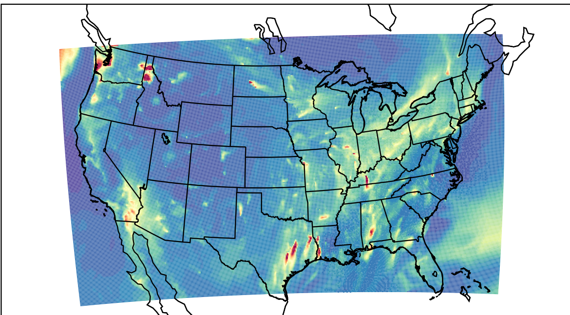
WRF 2019-11-15_06:00:00
