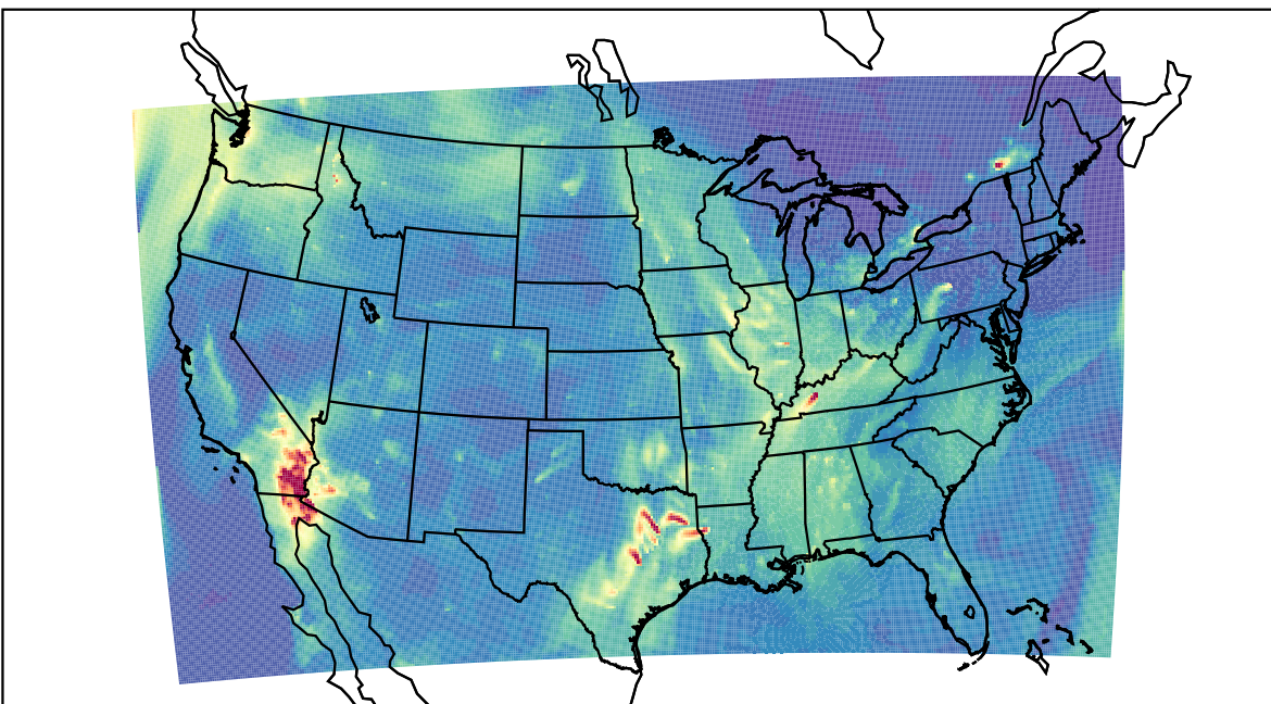
WRF 2019-11-16_13:00:00
