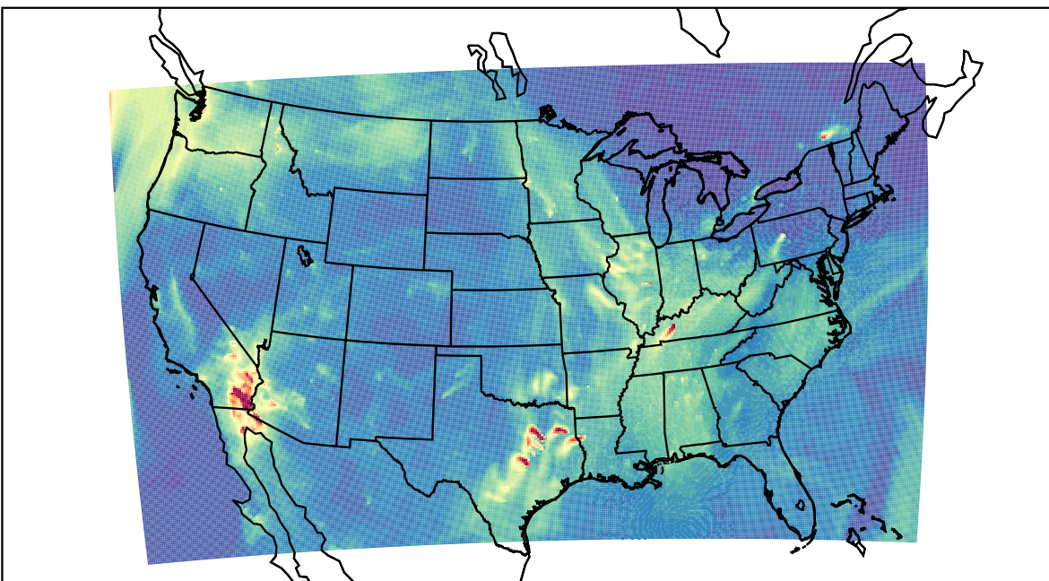
WRF 2019-11-16_11:00:00
