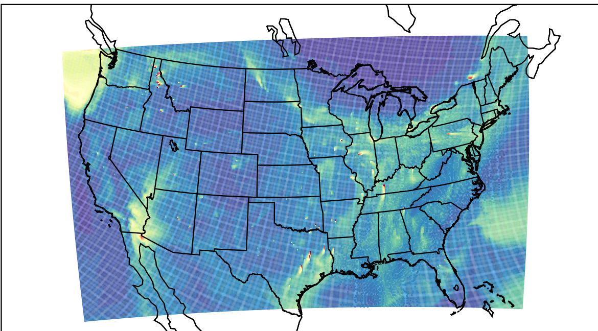
WRF 2019-11-15_20:00:00
