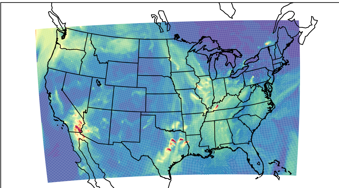
WRF 2019-11-16_10:00:00
