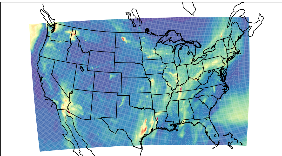
WRF 2019-11-15_11:00:00
