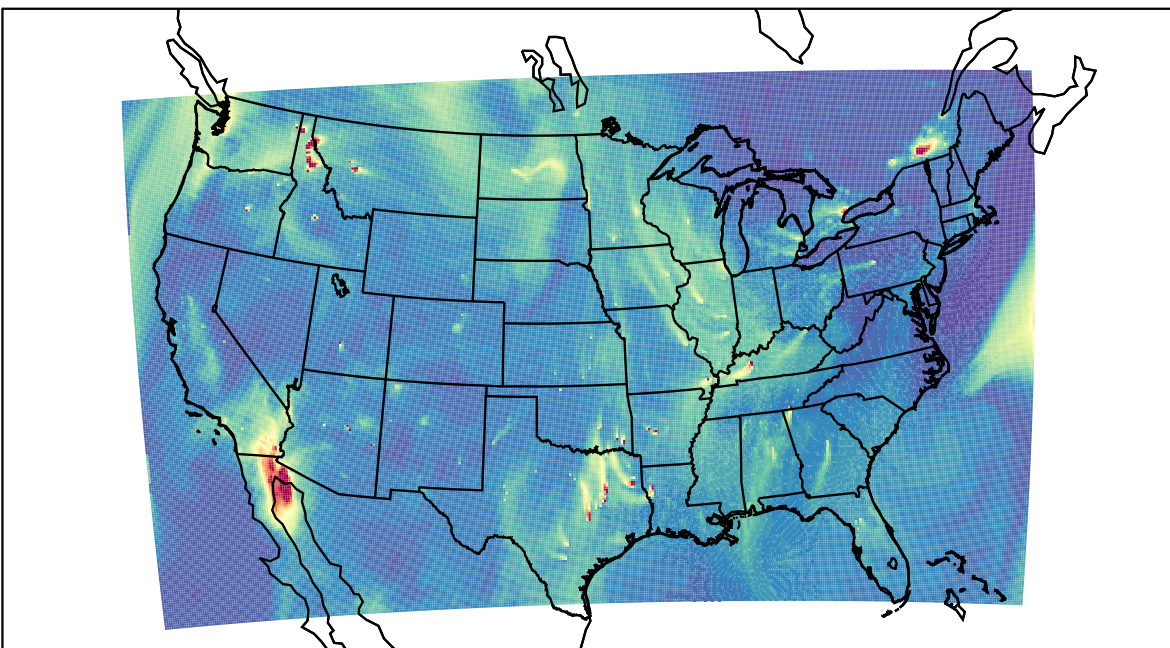
WRF 2019-11-16_21:00:00
