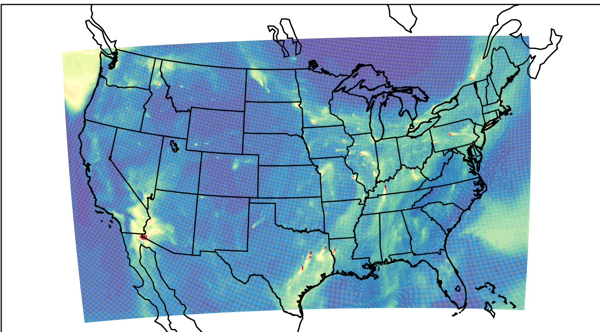
WRF 2019-11-15_17:00:00
