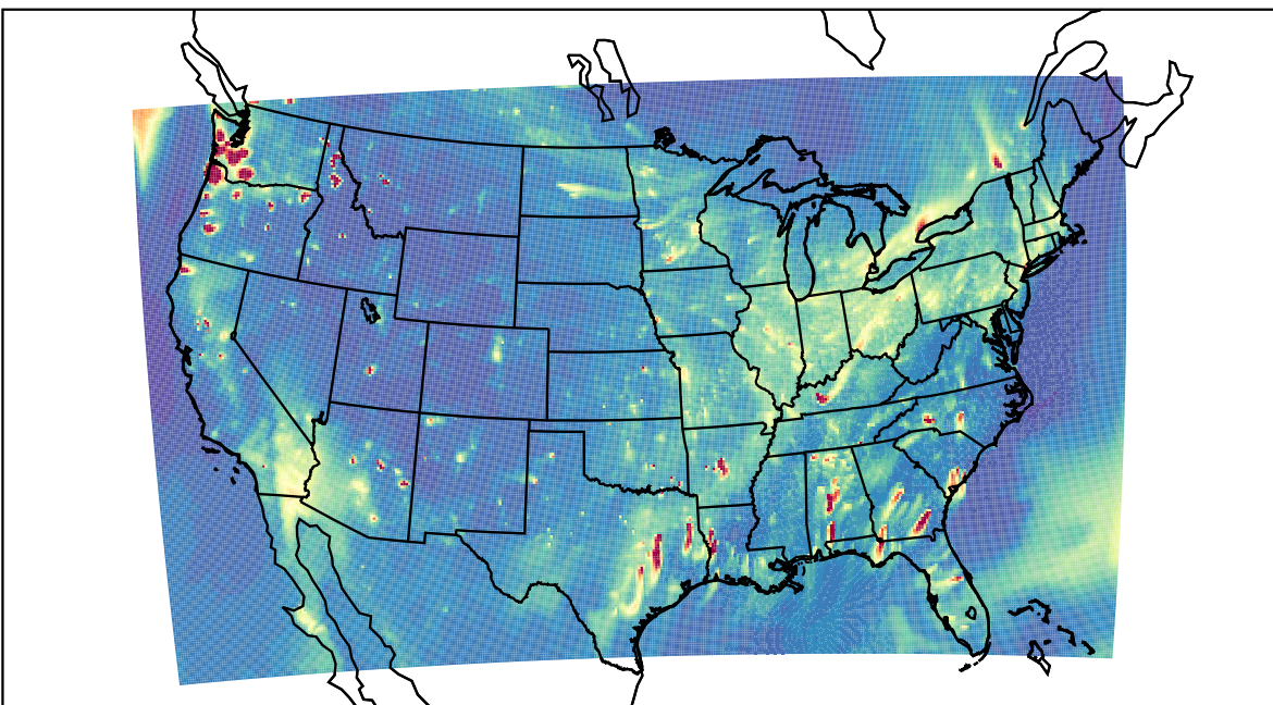
WRF 2019-11-15_01:00:00
