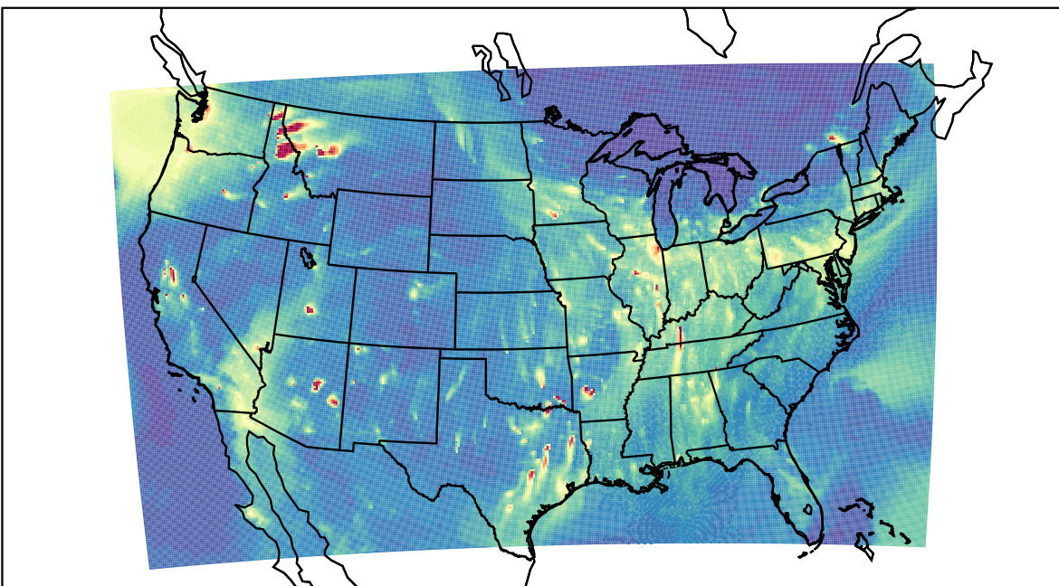
WRF 2019-11-16_02:00:00
