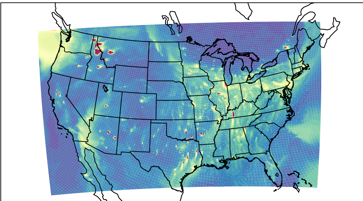
WRF 2019-11-16_00:00:00
