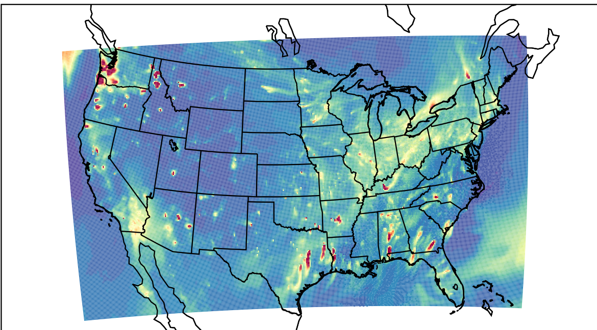
WRF 2019-11-15_02:00:00
