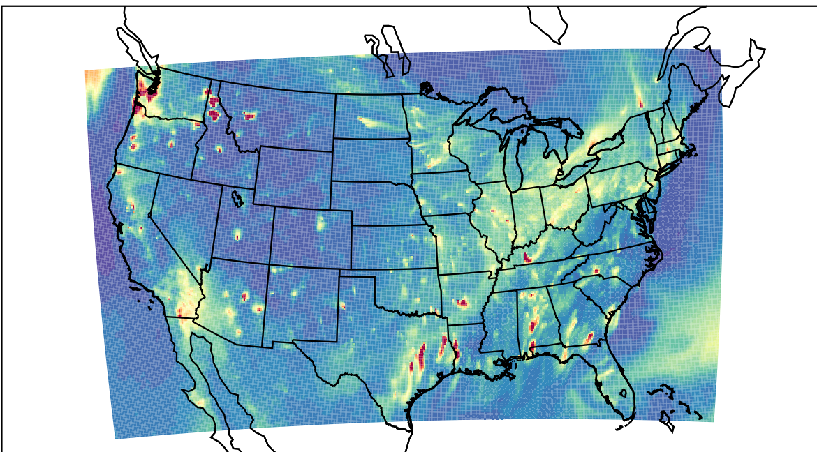
WRF 2019-11-15_03:00:00
