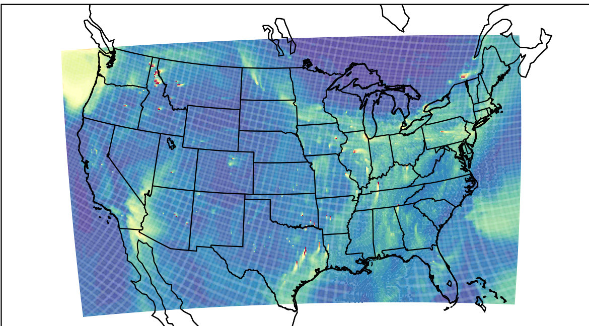
WRF 2019-11-15_21:00:00
