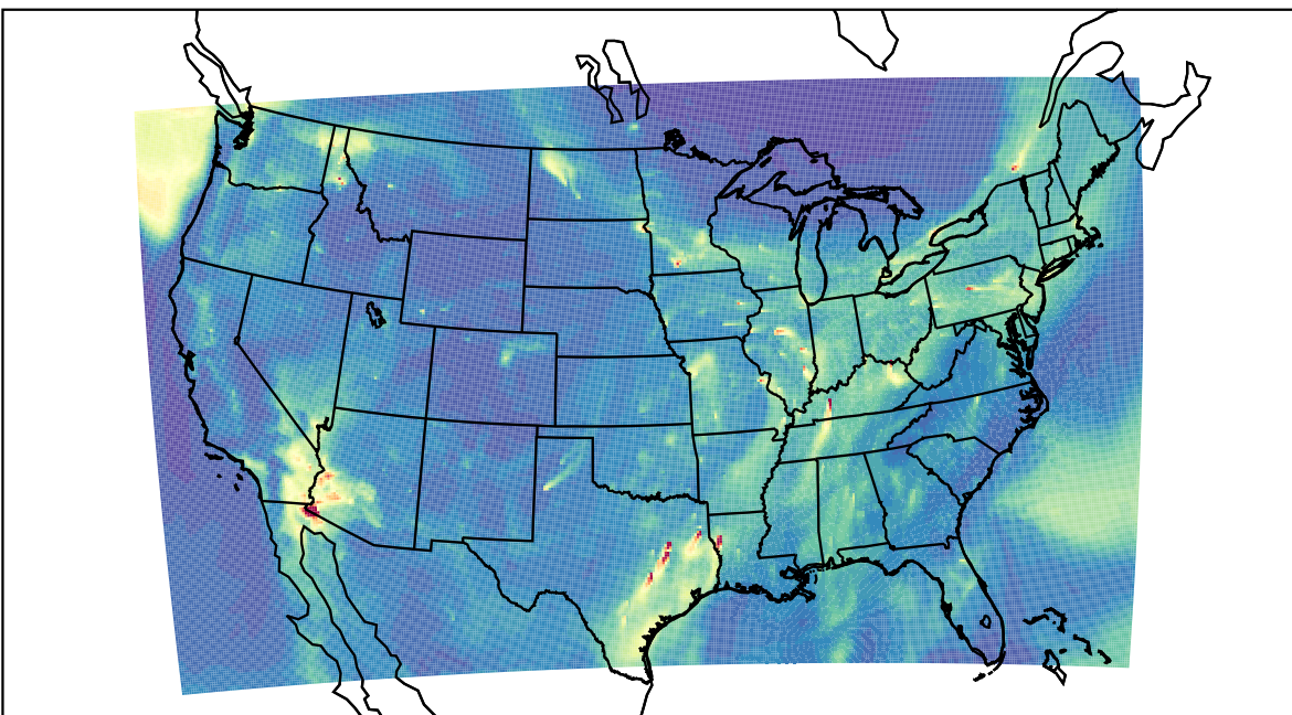
WRF 2019-11-15_16:00:00
