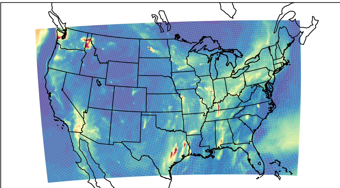
WRF 2019-11-15_08:00:00
