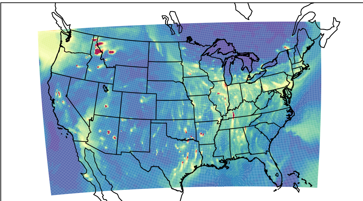
WRF 2019-11-16_01:00:00
