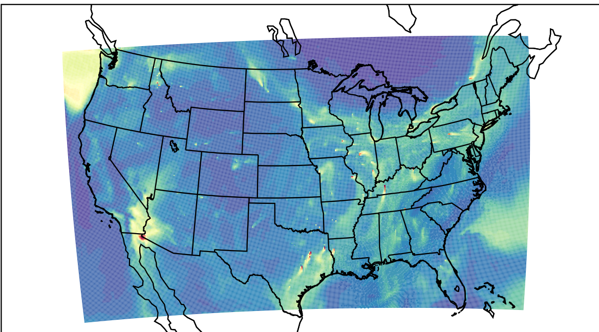
WRF 2019-11-15_18:00:00
