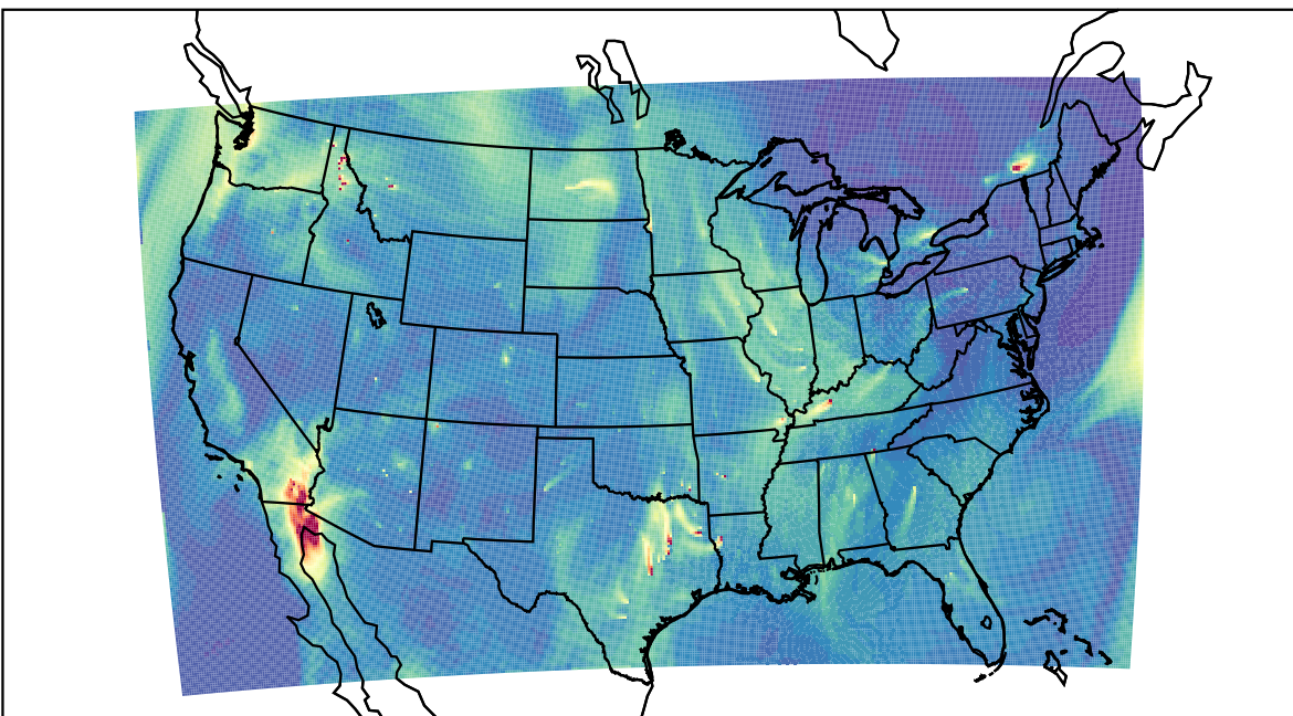
WRF 2019-11-16_19:00:00
