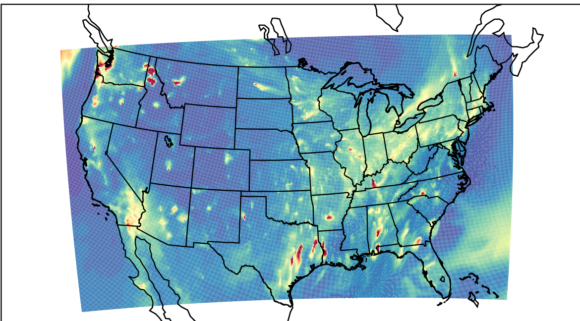
WRF 2019-11-15_04:00:00
