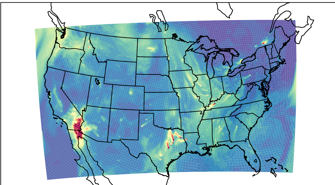
WRF 2019-11-16_16:00:00
