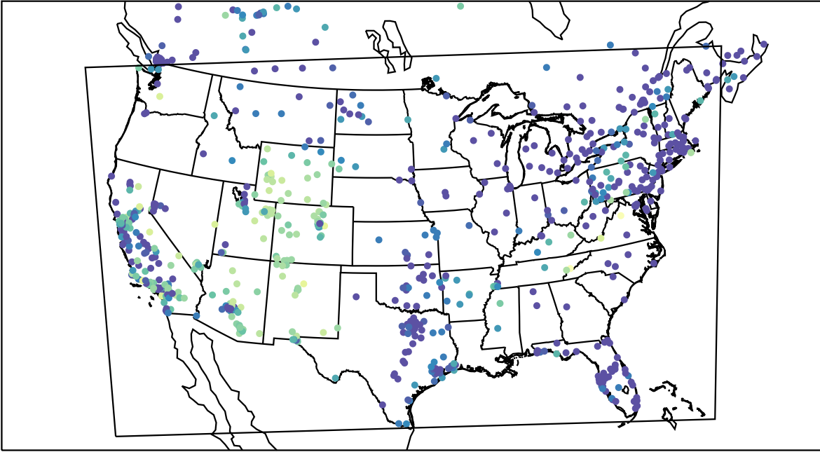
AirNOW (2019-11-26_12:00:00)
