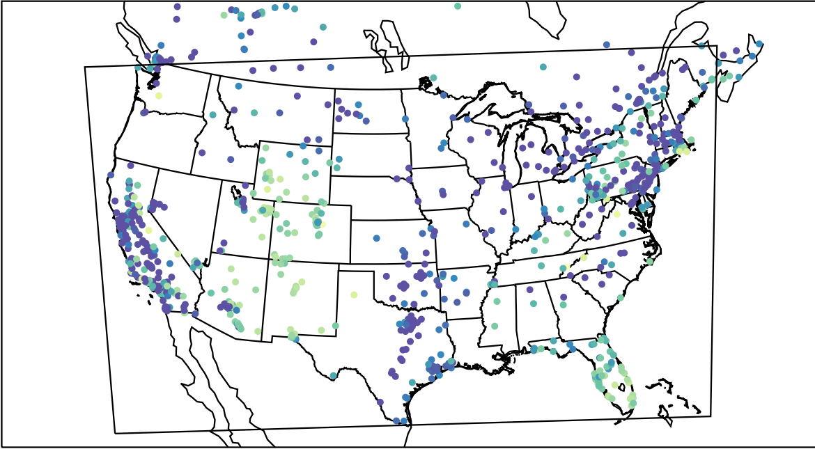
AirNOW (2019-11-26_15:00:00)
