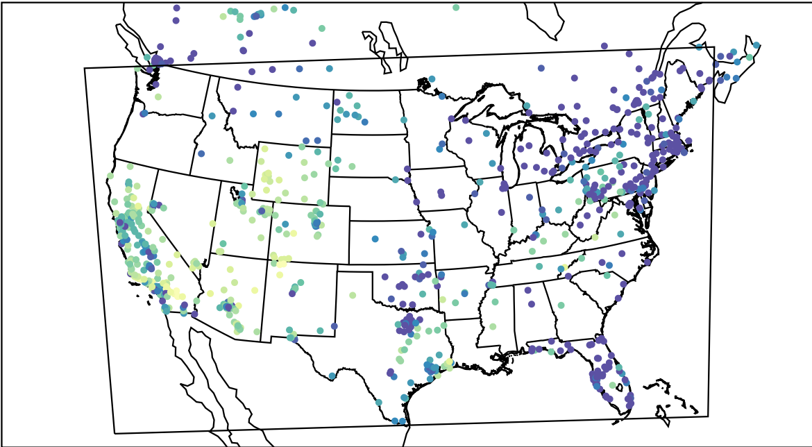
AirNOW (2019-11-26_03:00:00)
