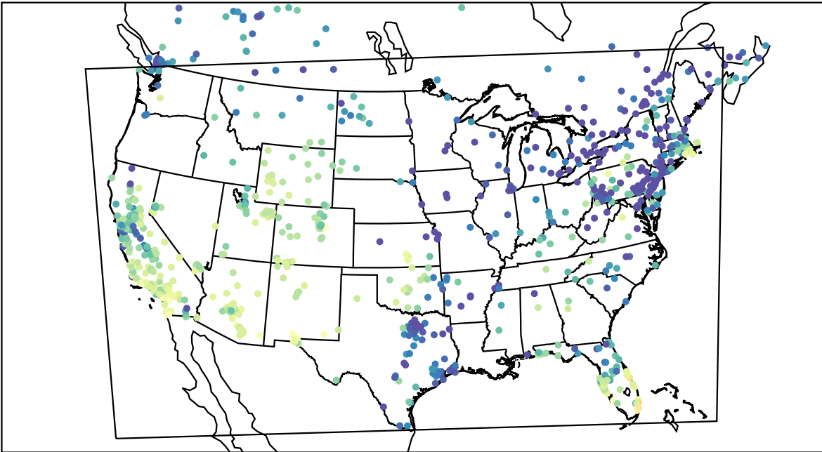
AirNOW (2019-11-26_22:00:00)
