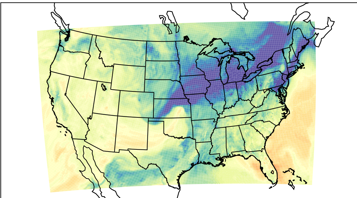
WRF (2019-11-26_22:00:00)
