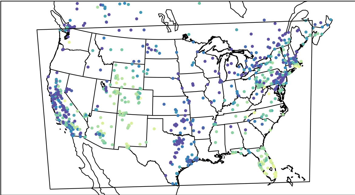
AirNOW (2019-11-26_16:00:00)
