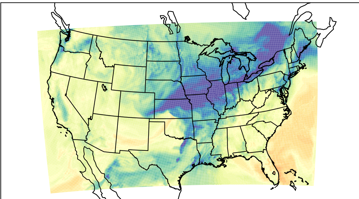
WRF (2019-11-26_19:00:00)
