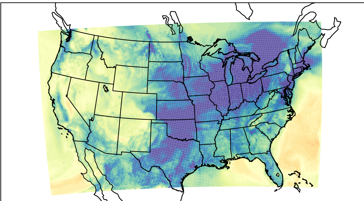
WRF (2019-11-26_13:00:00)
