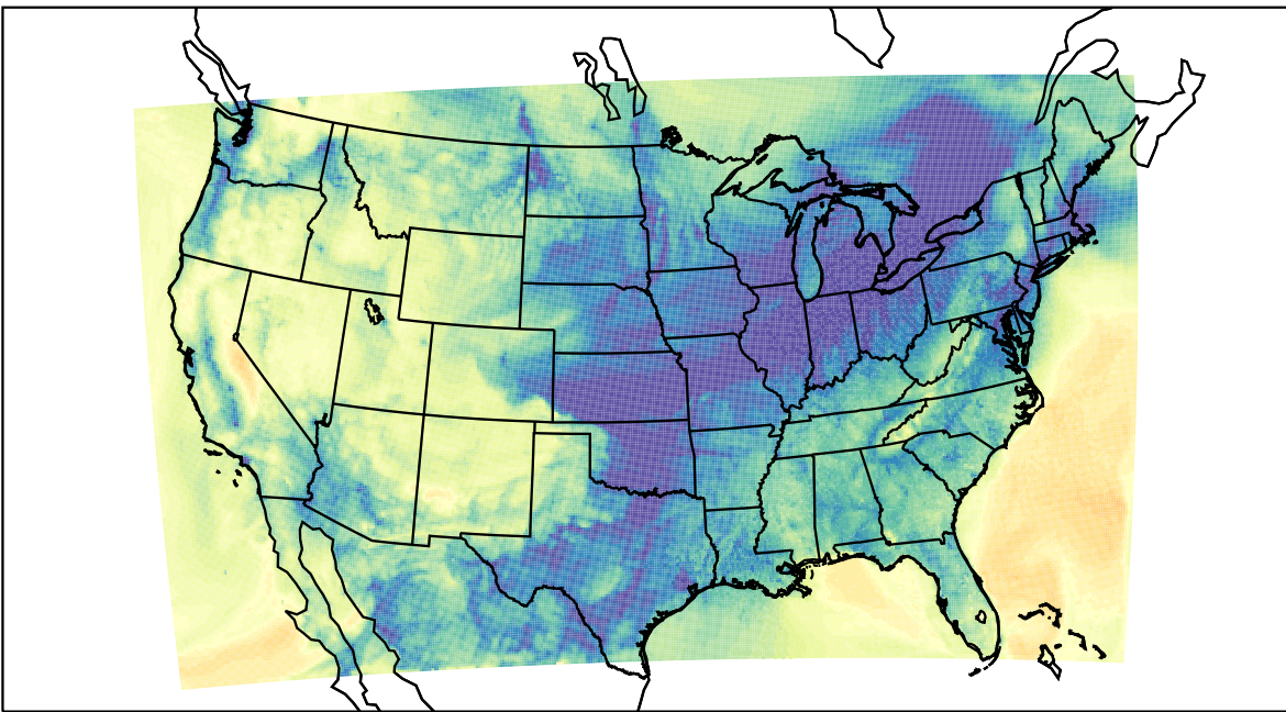
WRF (2019-11-26_15:00:00)
