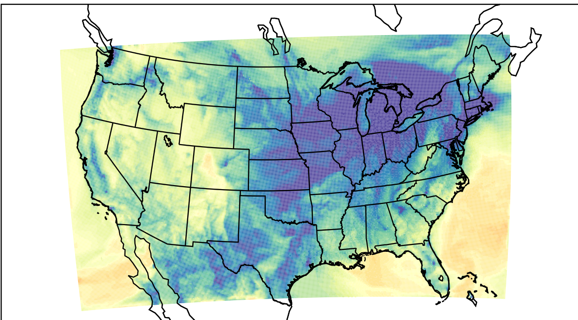
WRF (2019-11-26_06:00:00)
