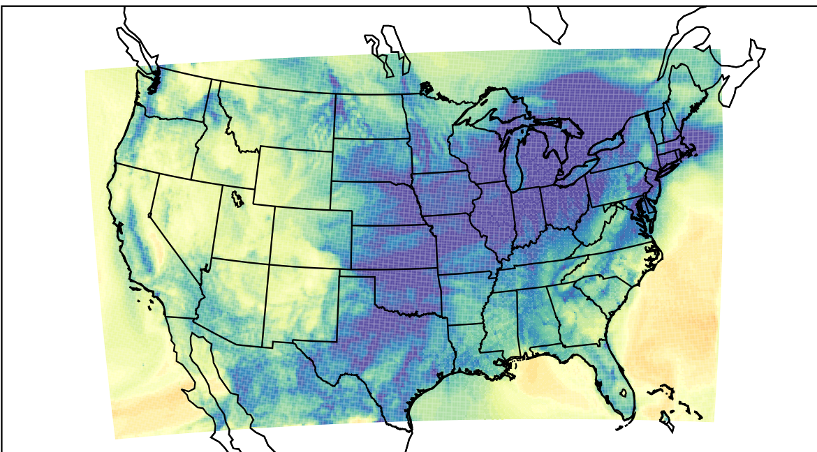
WRF (2019-11-26_11:00:00)
