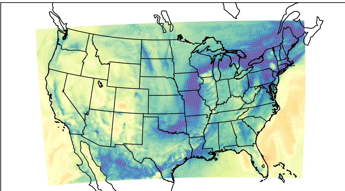
WRF (2019-11-27_08:00:00)
