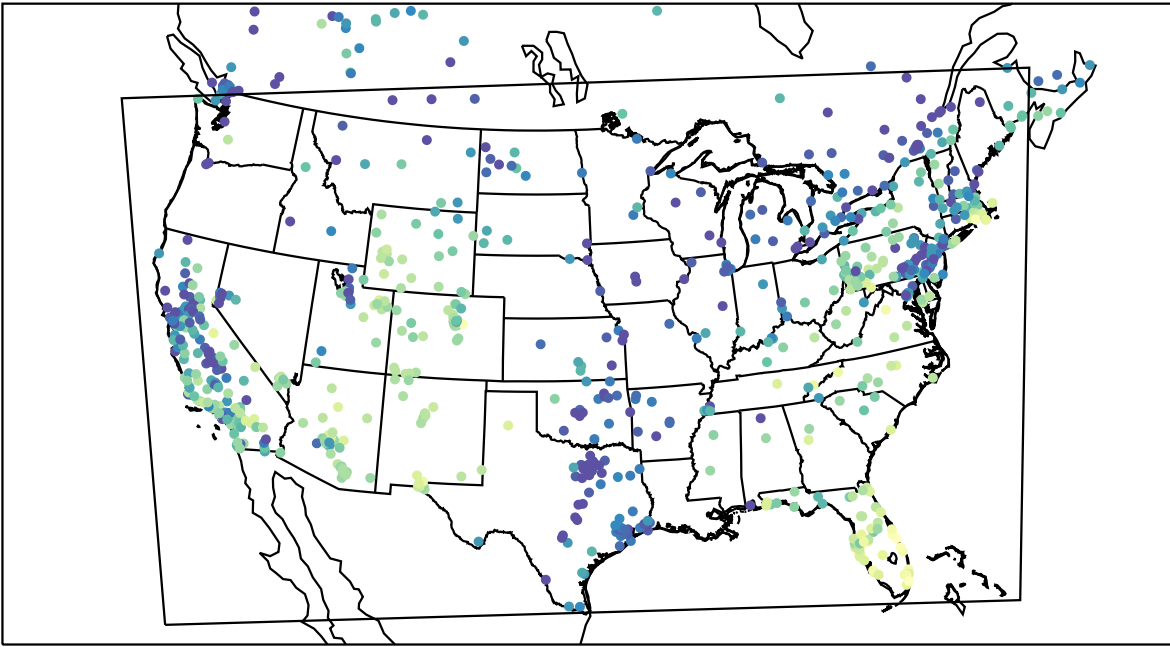
AirNOW (2019-11-26_17:00:00)
