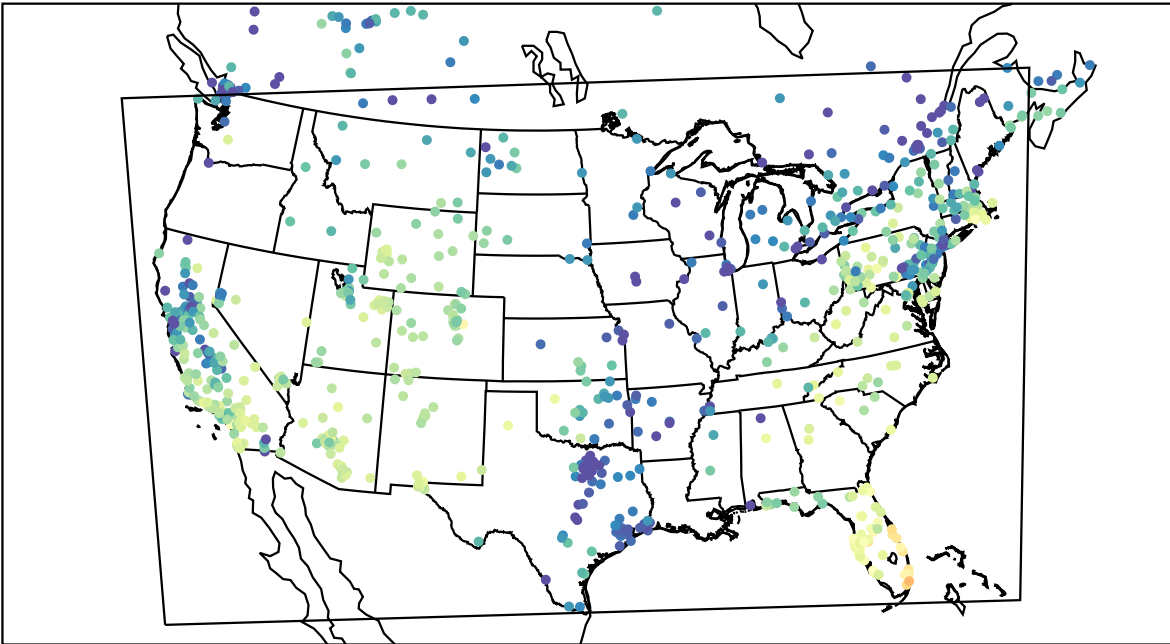
AirNOW (2019-11-26_19:00:00)
