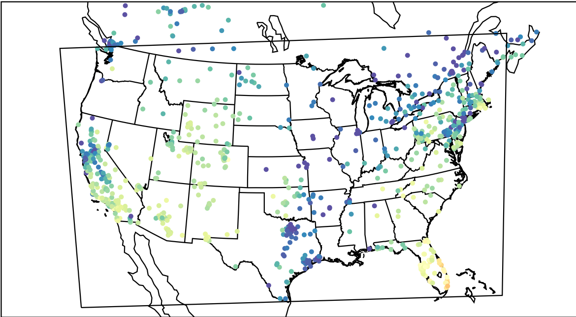
AirNOW (2019-11-26_20:00:00)
