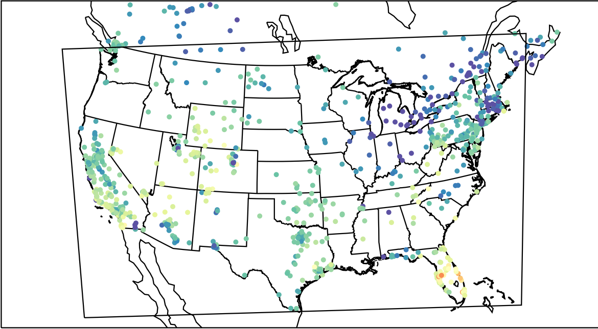
AirNOW (2019-11-27_20:00:00)
