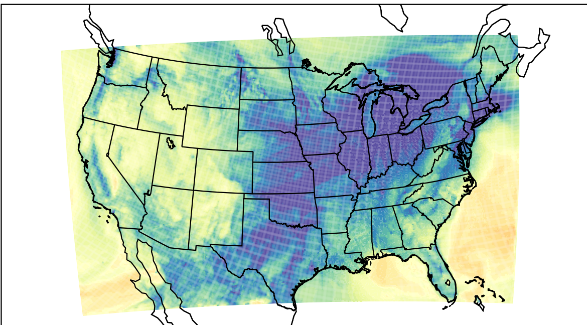
WRF (2019-11-26_10:00:00)
