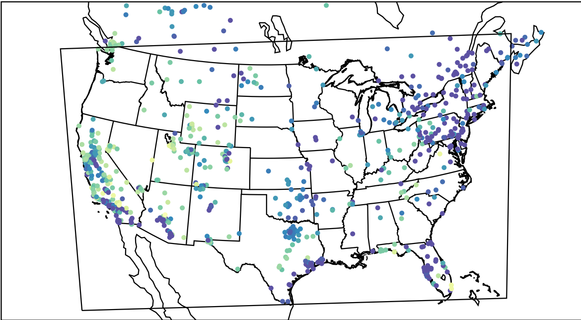
AirNOW (2019-11-27_08:00:00)
