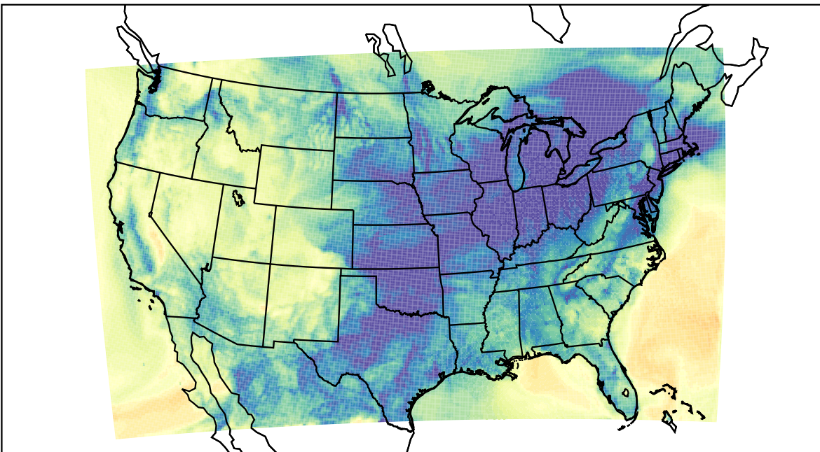
WRF (2019-11-26_12:00:00)
