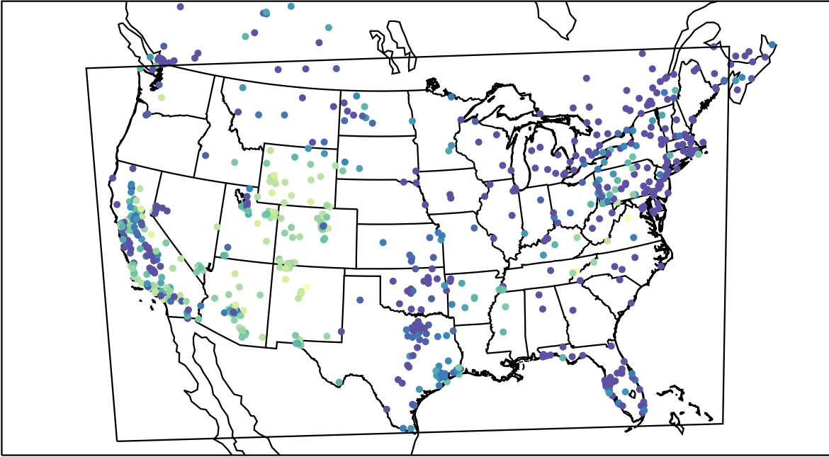
AirNOW (2019-11-26_10:00:00)
