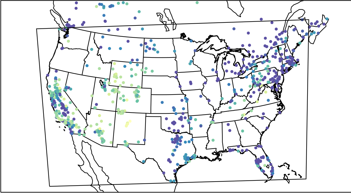
AirNOW (2019-11-26_08:00:00)
