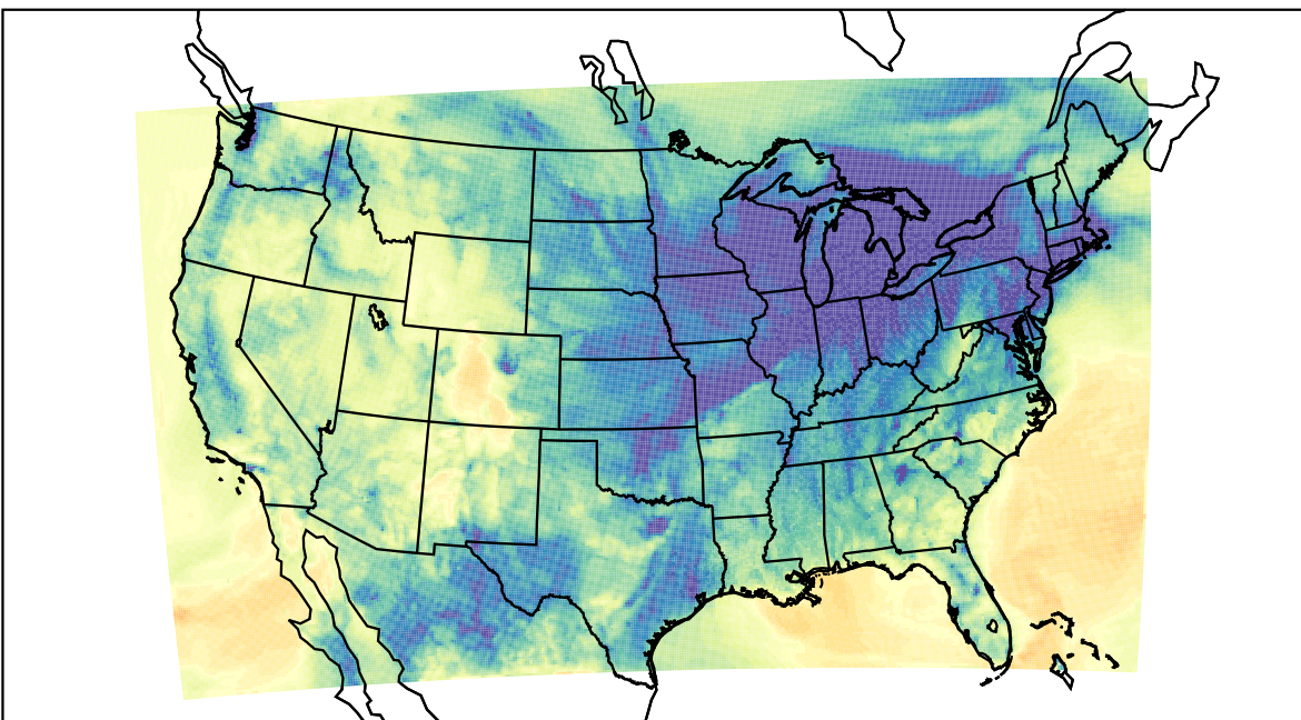
WRF (2019-11-26_03:00:00)
