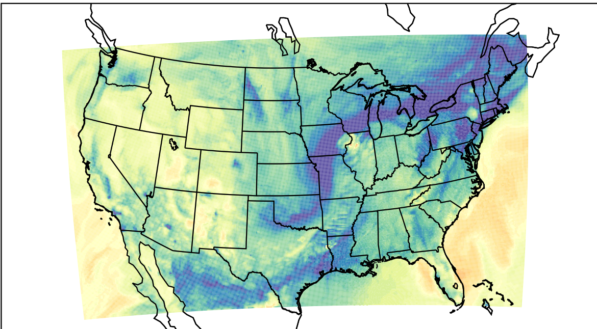
WRF (2019-11-27_06:00:00)
