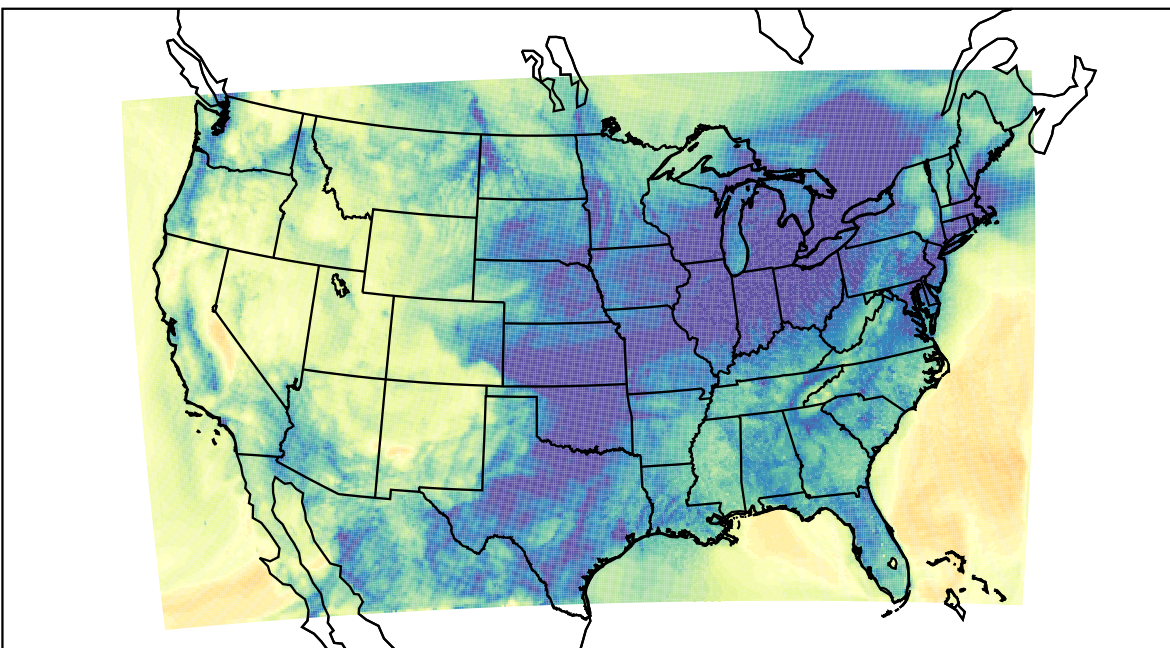
WRF (2019-11-26_14:00:00)
