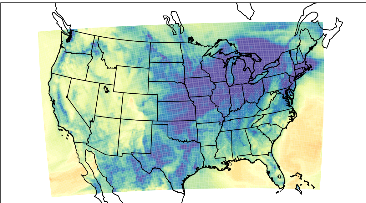
WRF (2019-11-26_07:00:00)
