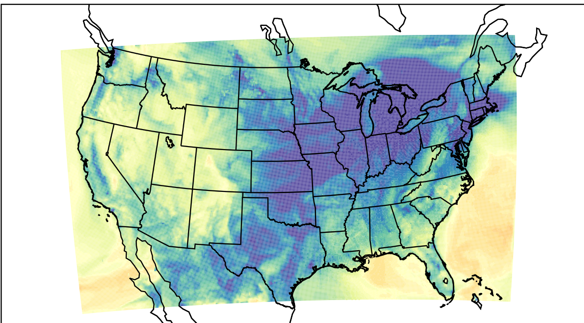
WRF (2019-11-26_08:00:00)
