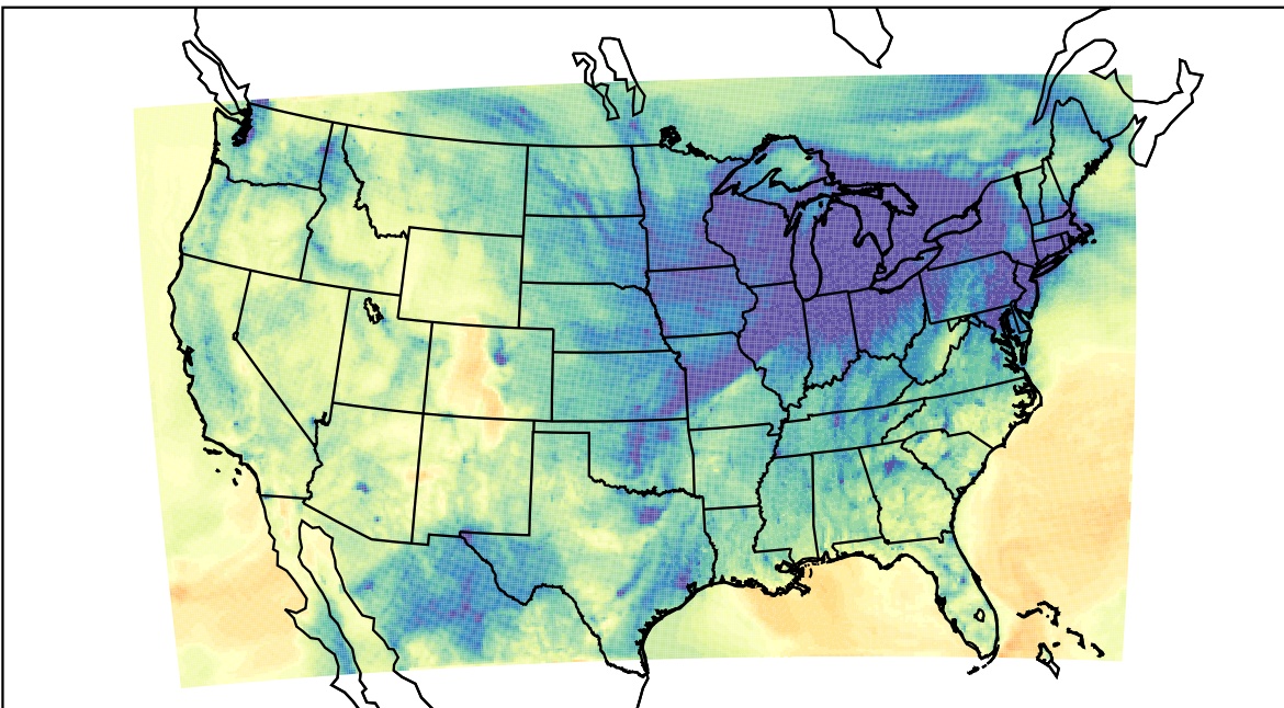
WRF (2019-11-26_01:00:00)
