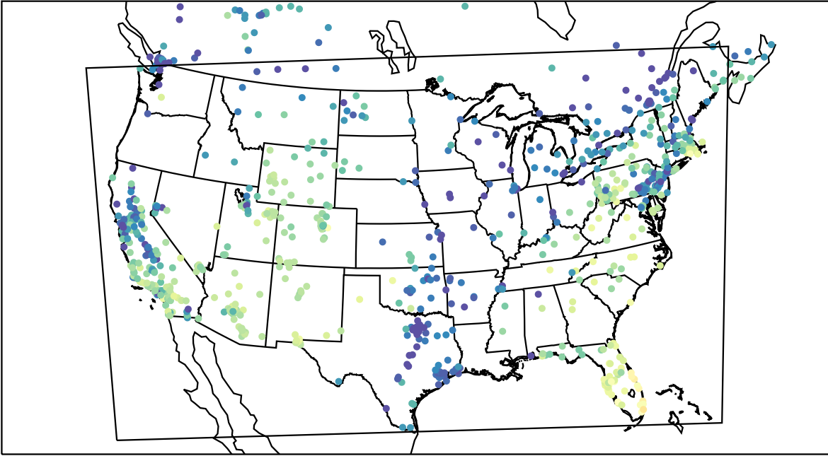
AirNOW (2019-11-26_18:00:00)
