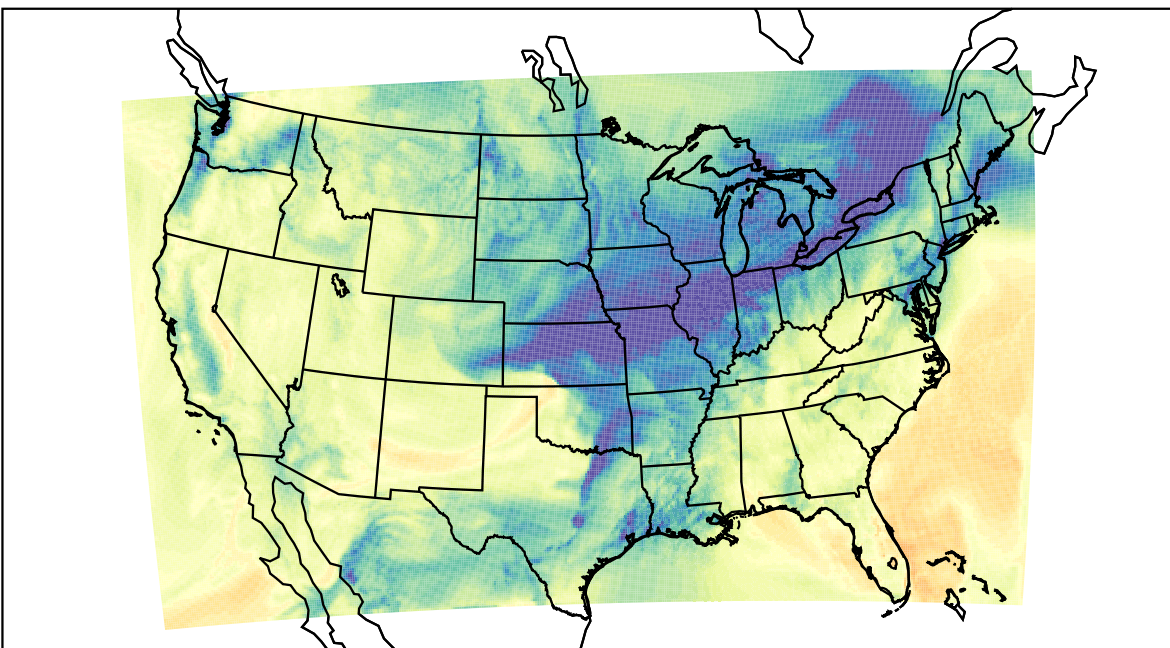
WRF (2019-11-26_18:00:00)
