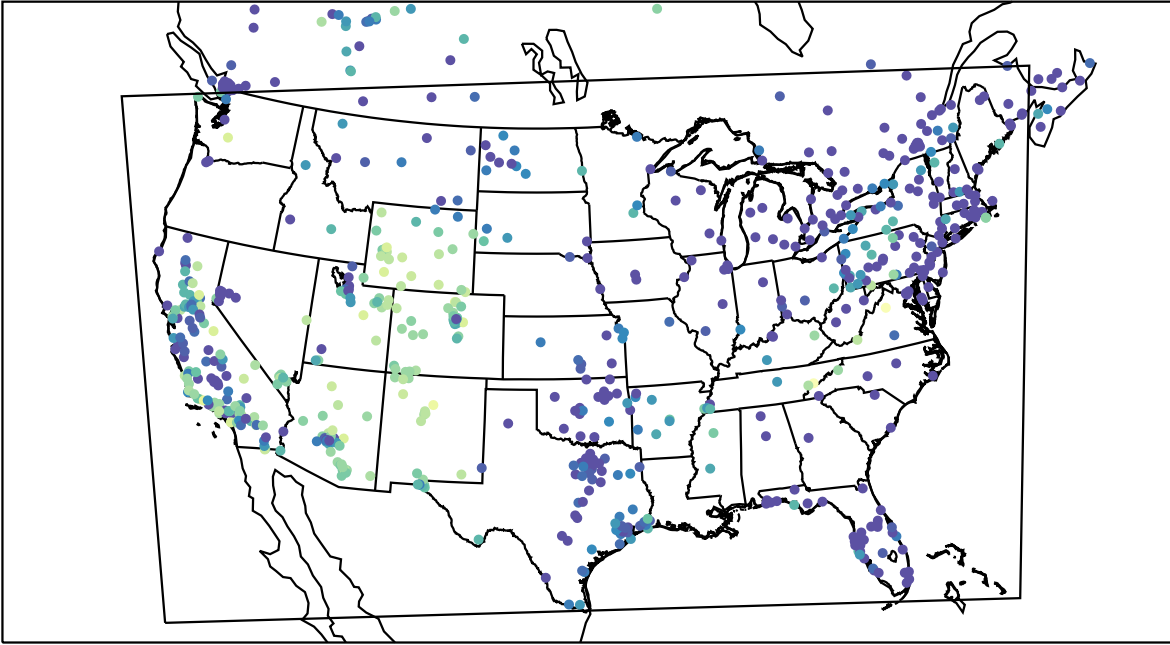
AirNOW (2019-11-26_11:00:00)
