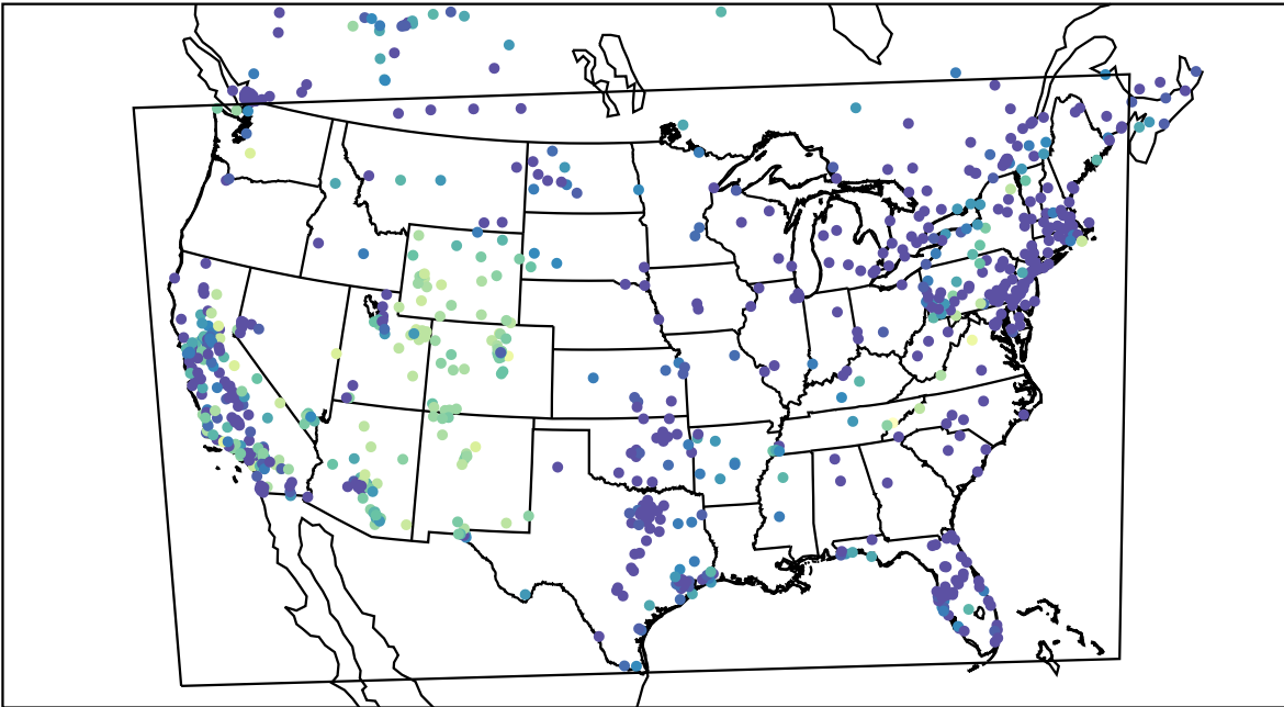
AirNOW (2019-11-26_13:00:00)
