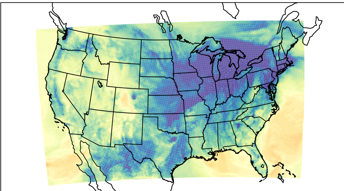
WRF (2019-11-26_04:00:00)
