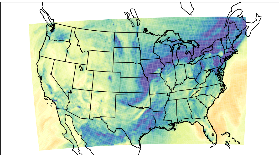
WRF (2019-11-27_04:00:00)
