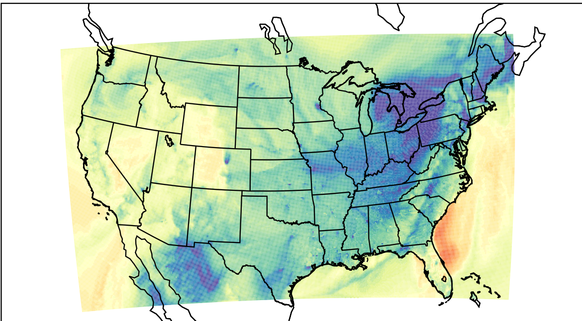
WRF (2019-11-27_23:00:00)
