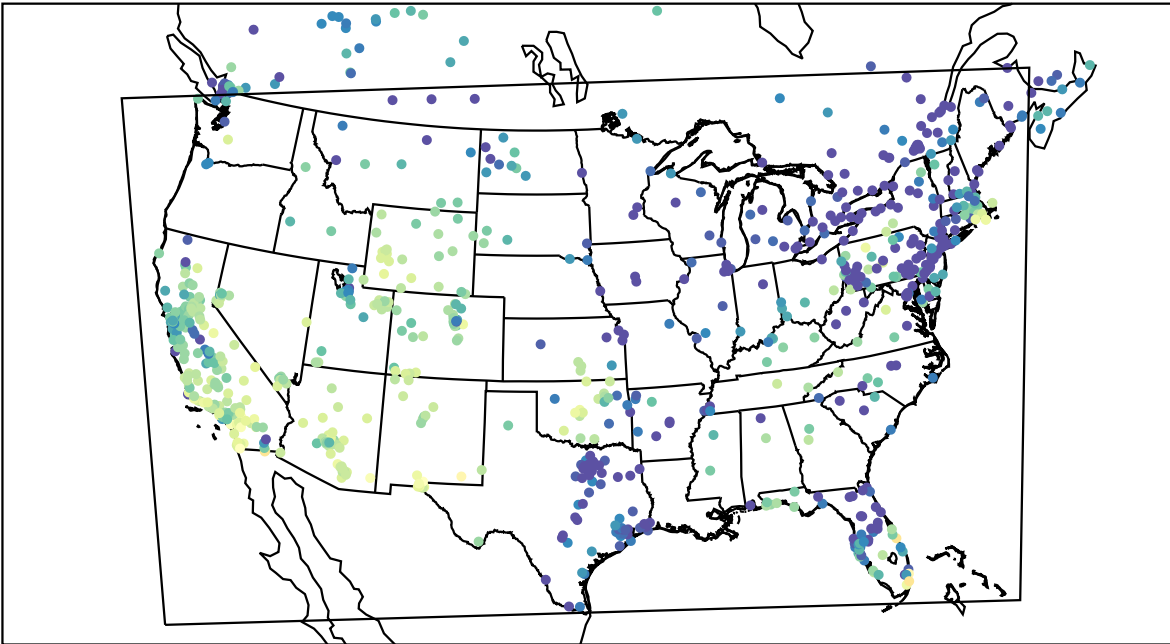
AirNOW (2019-11-26_23:00:00)
