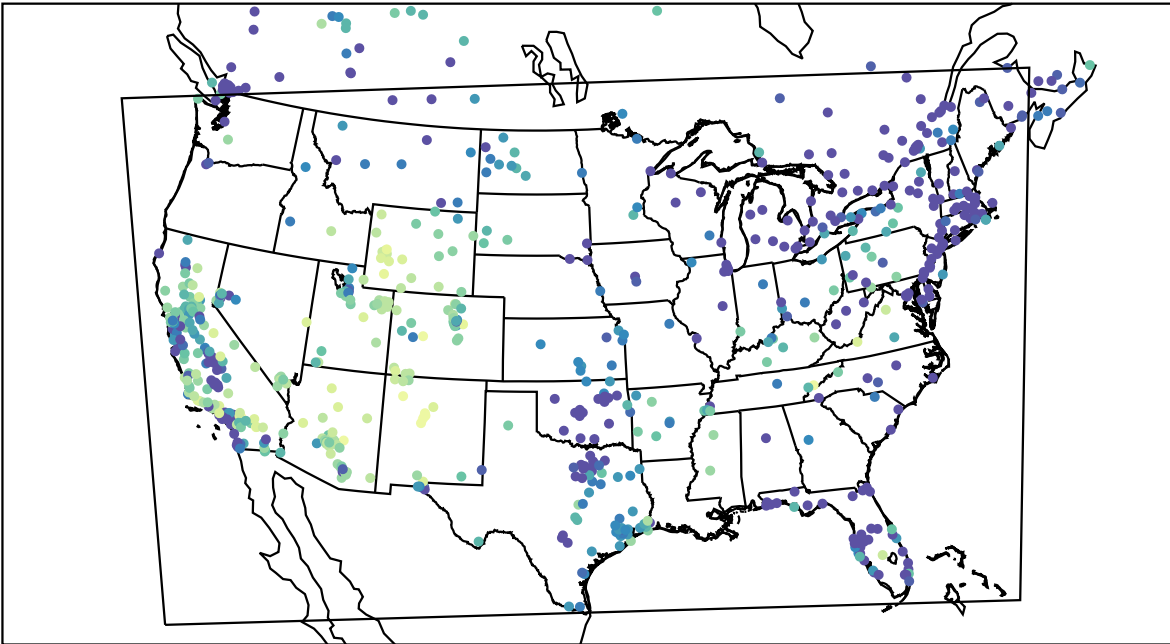
AirNOW (2019-11-26_06:00:00)
