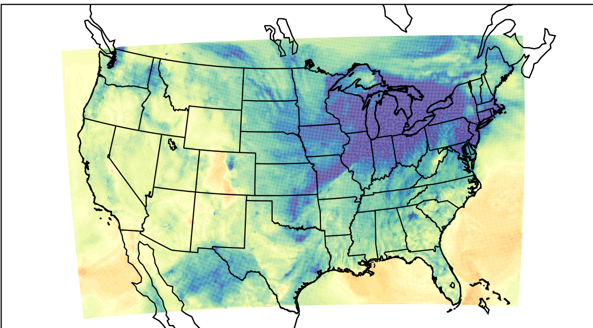
WRF (2019-11-26_00:00:00)
