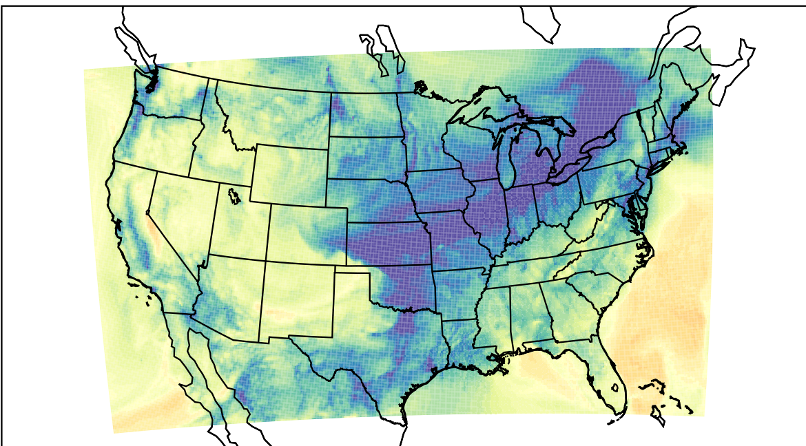
WRF (2019-11-26_16:00:00)
