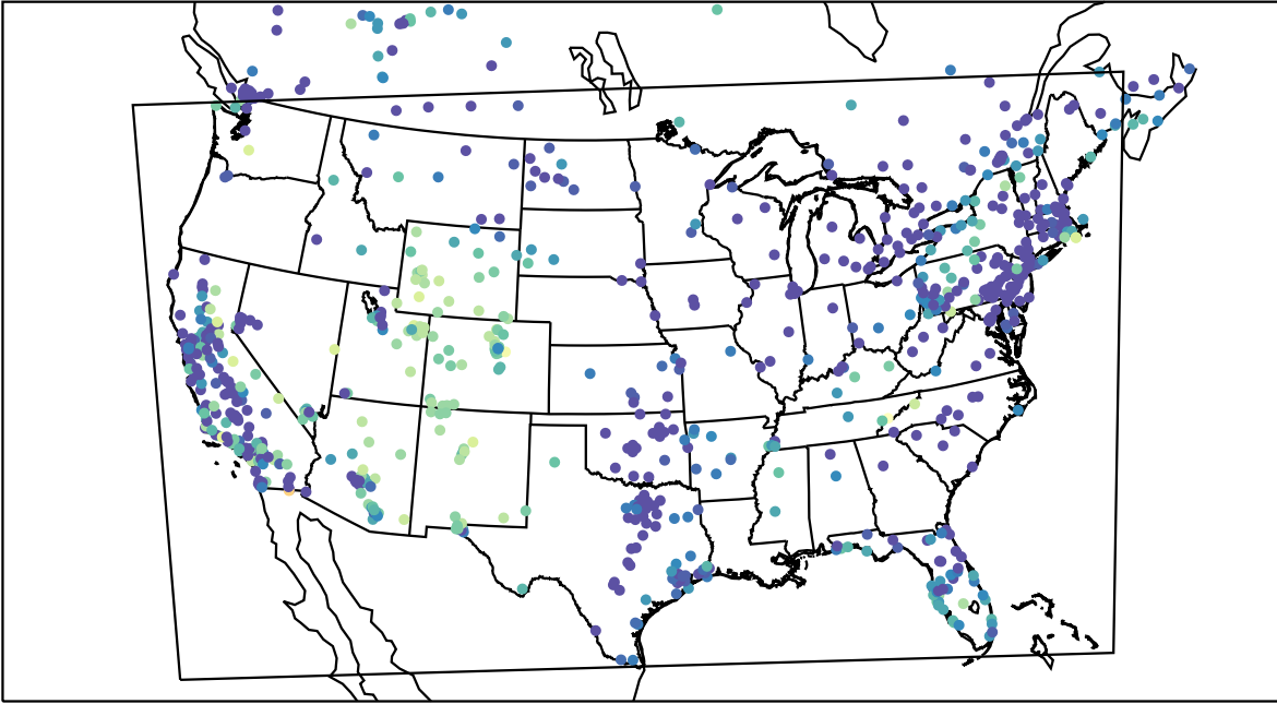
AirNOW (2019-11-26_14:00:00)
