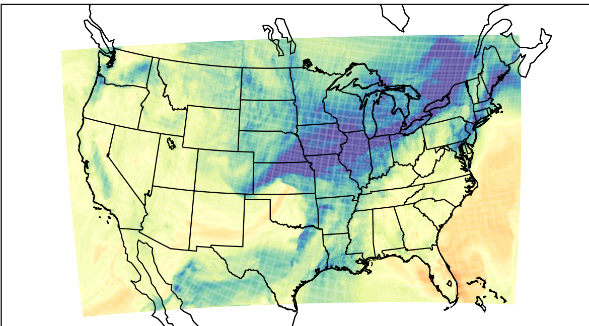
WRF (2019-11-26_20:00:00)
