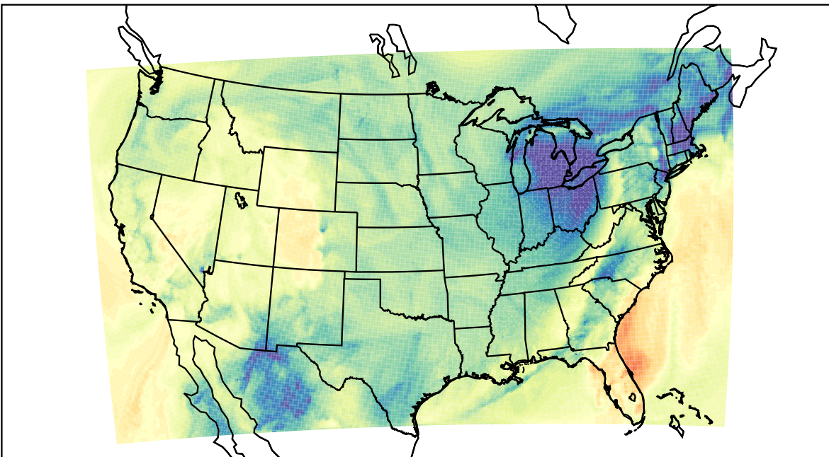
WRF (2019-11-27_20:00:00)
