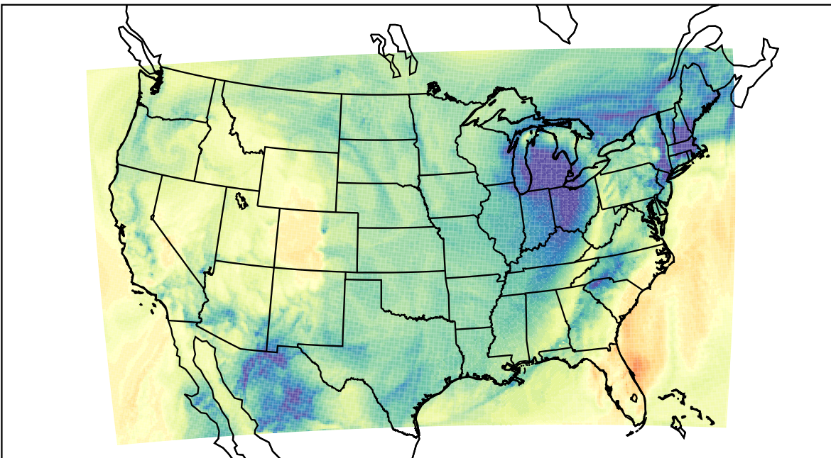
WRF (2019-11-27_18:00:00)
