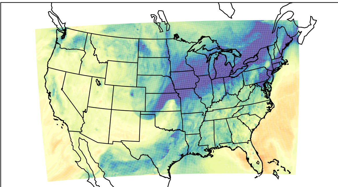
WRF (2019-11-26_23:00:00)
