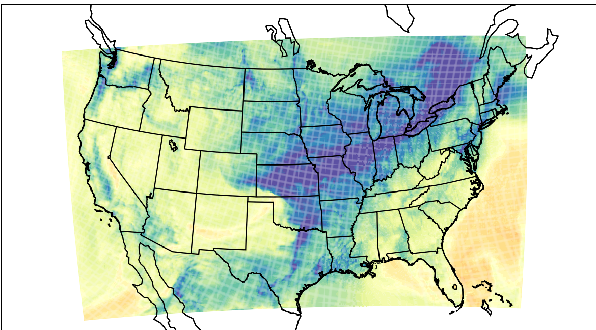
WRF (2019-11-26_17:00:00)
