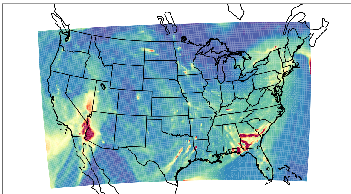
WRF 2019-11-28_03:00:00
