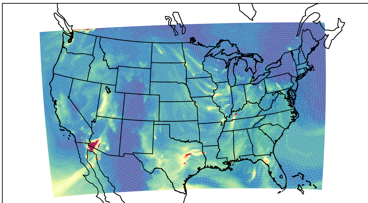
WRF 2019-11-29_09:00:00
