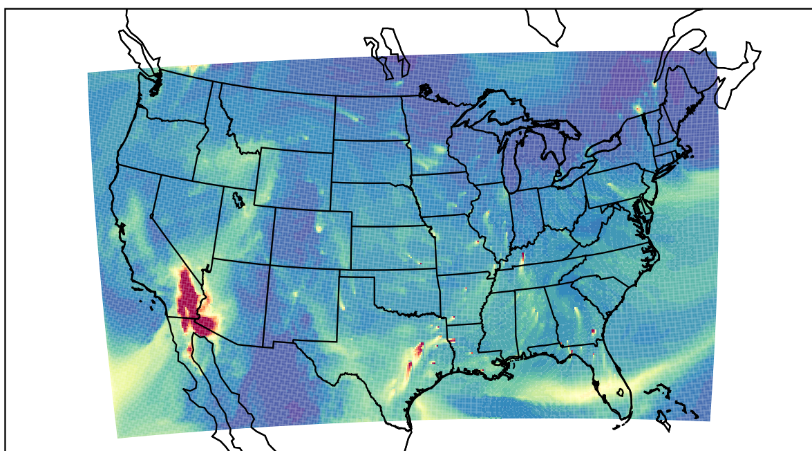
WRF 2019-11-28_20:00:00
