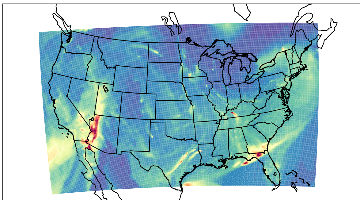
WRF 2019-11-28_08:00:00
