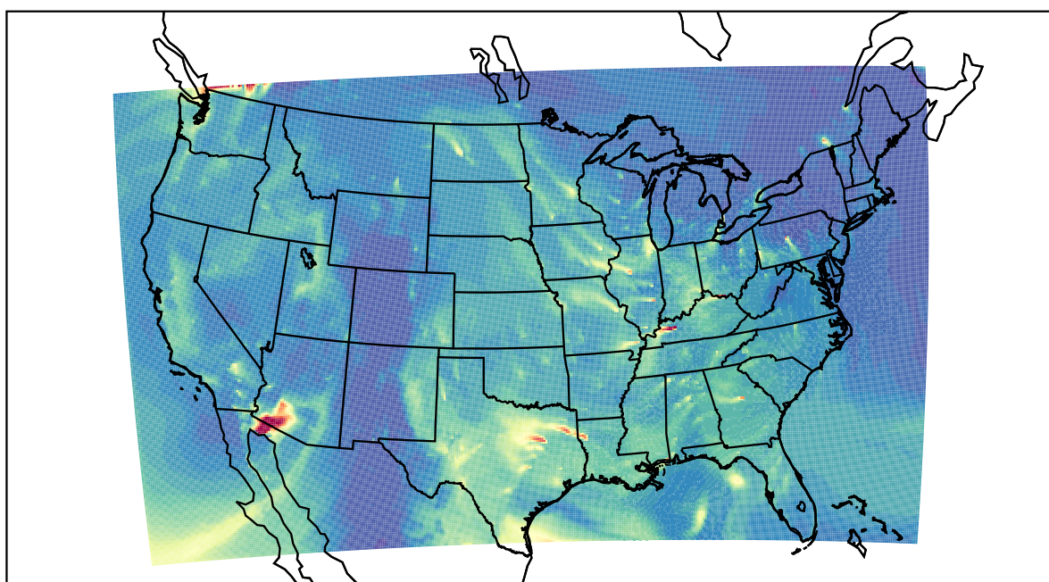
WRF 2019-11-29_15:00:00
