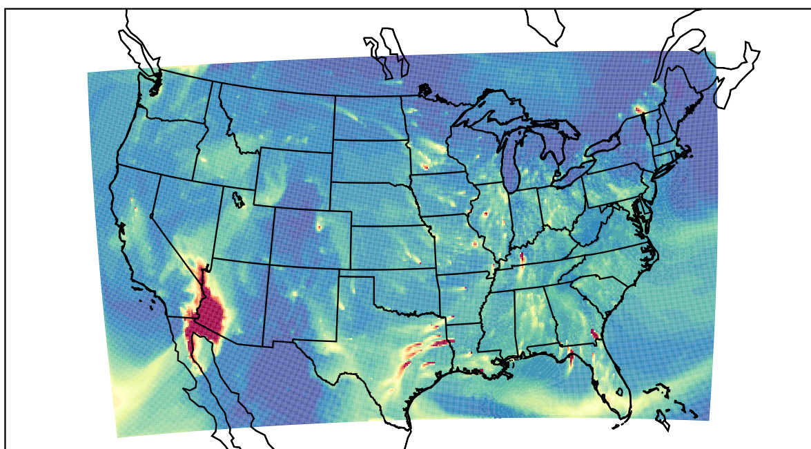
WRF 2019-11-29_01:00:00
