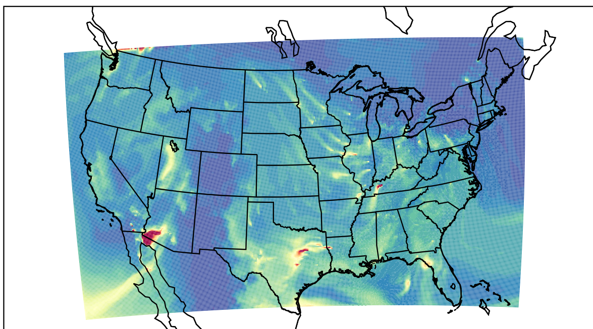
WRF 2019-11-29_10:00:00
