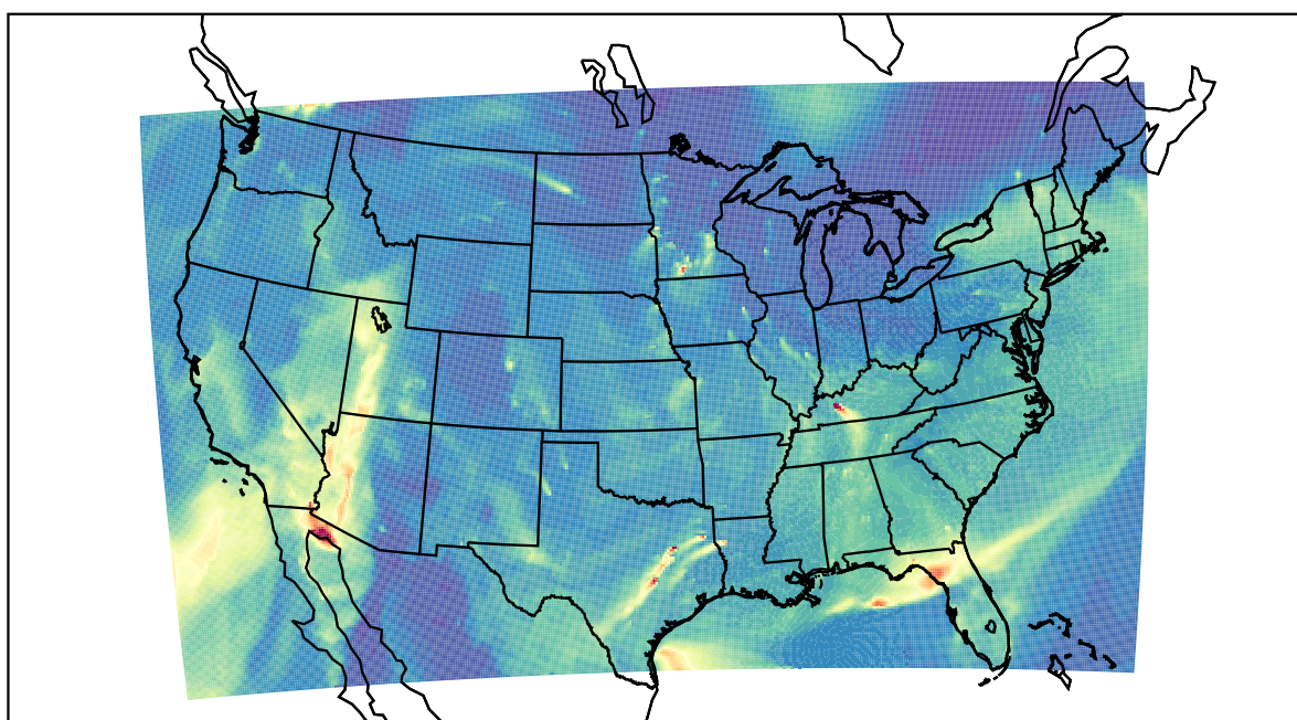
WRF 2019-11-28_11:00:00
