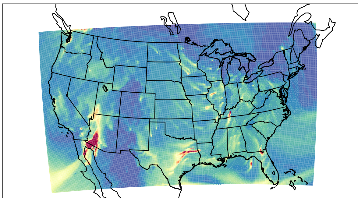
WRF 2019-11-29_05:00:00
