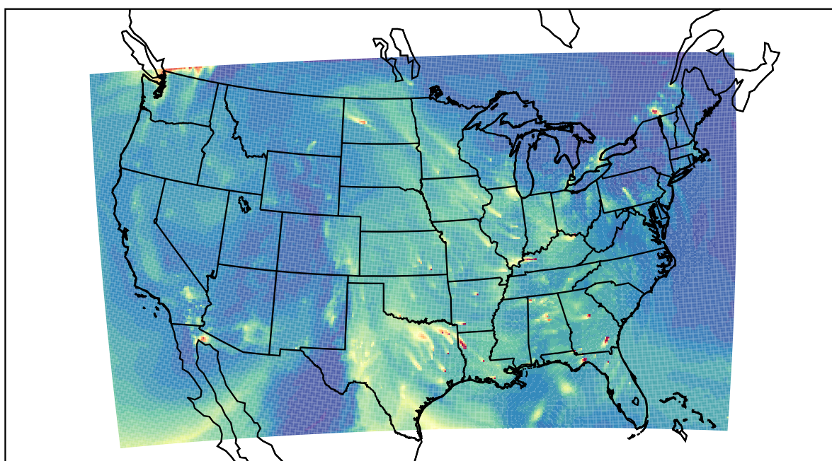
WRF 2019-11-29_21:00:00
