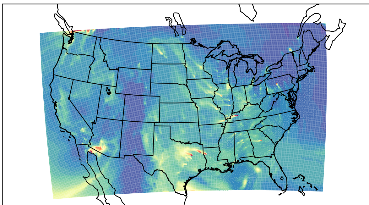
WRF 2019-11-29_16:00:00
