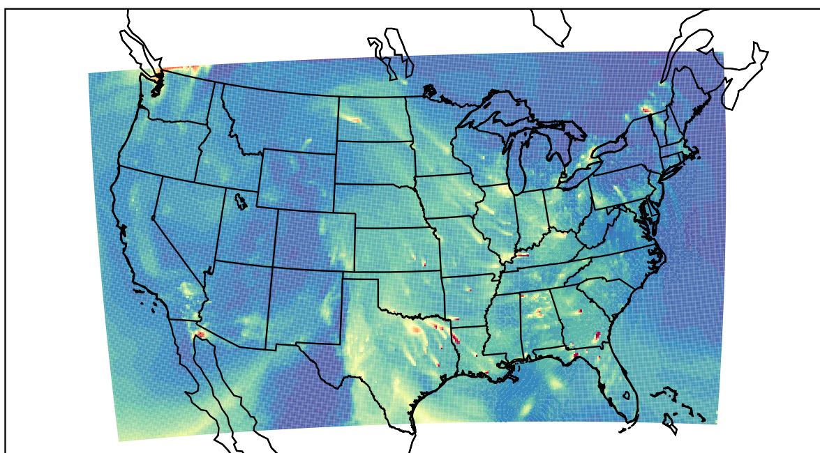
WRF 2019-11-29_22:00:00
