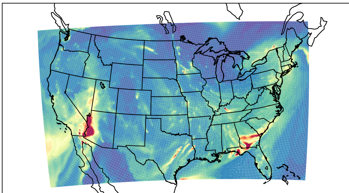
WRF 2019-11-28_05:00:00
