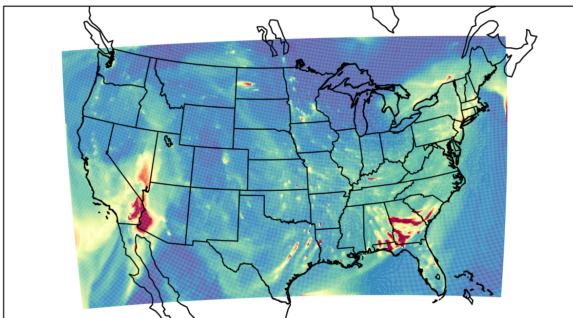
WRF 2019-11-28_02:00:00
