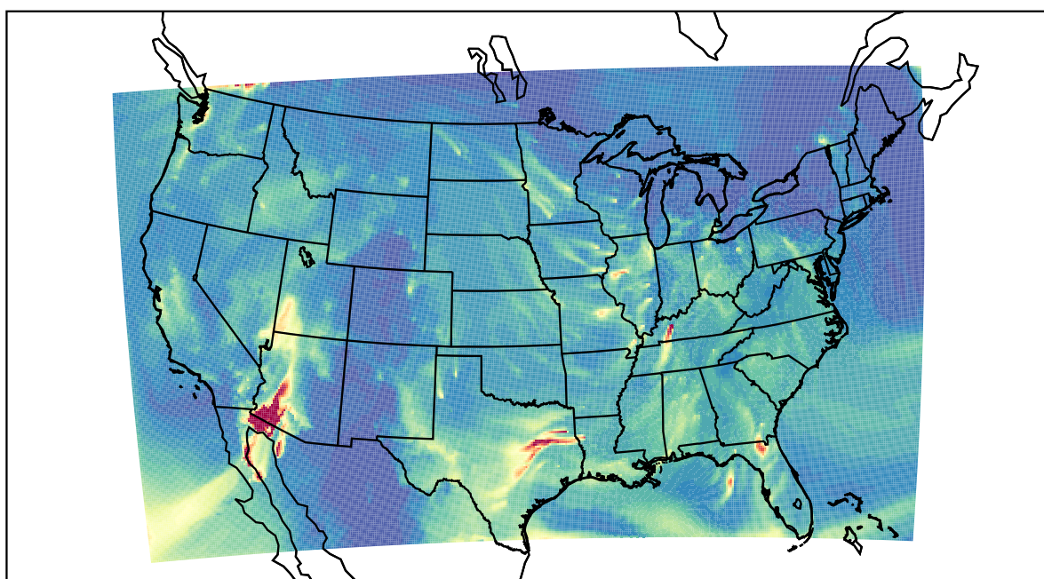
WRF 2019-11-29_06:00:00
