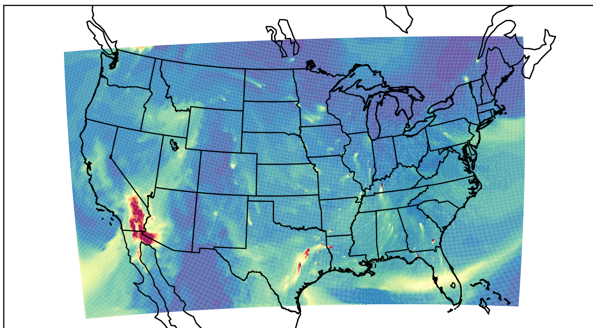
WRF 2019-11-28_19:00:00
