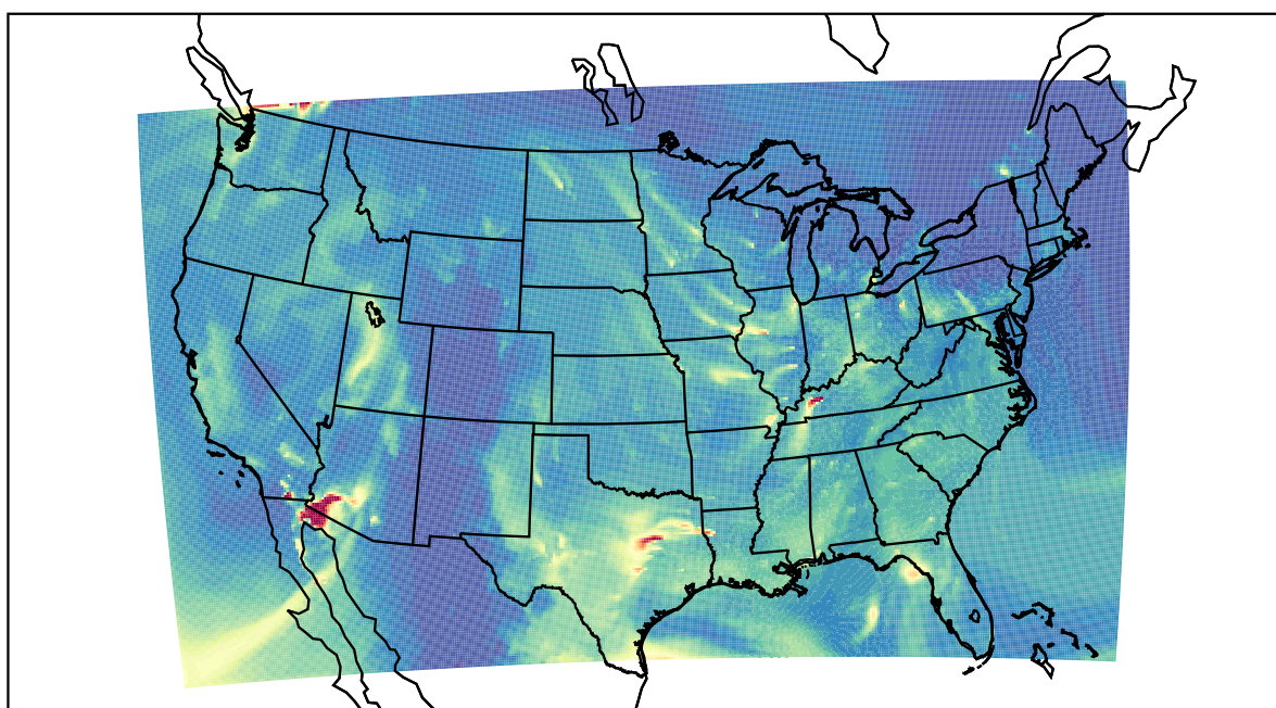
WRF 2019-11-29_11:00:00
