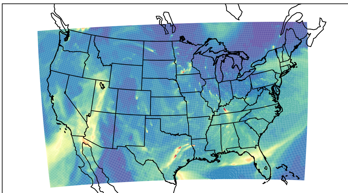
WRF 2019-11-28_13:00:00
