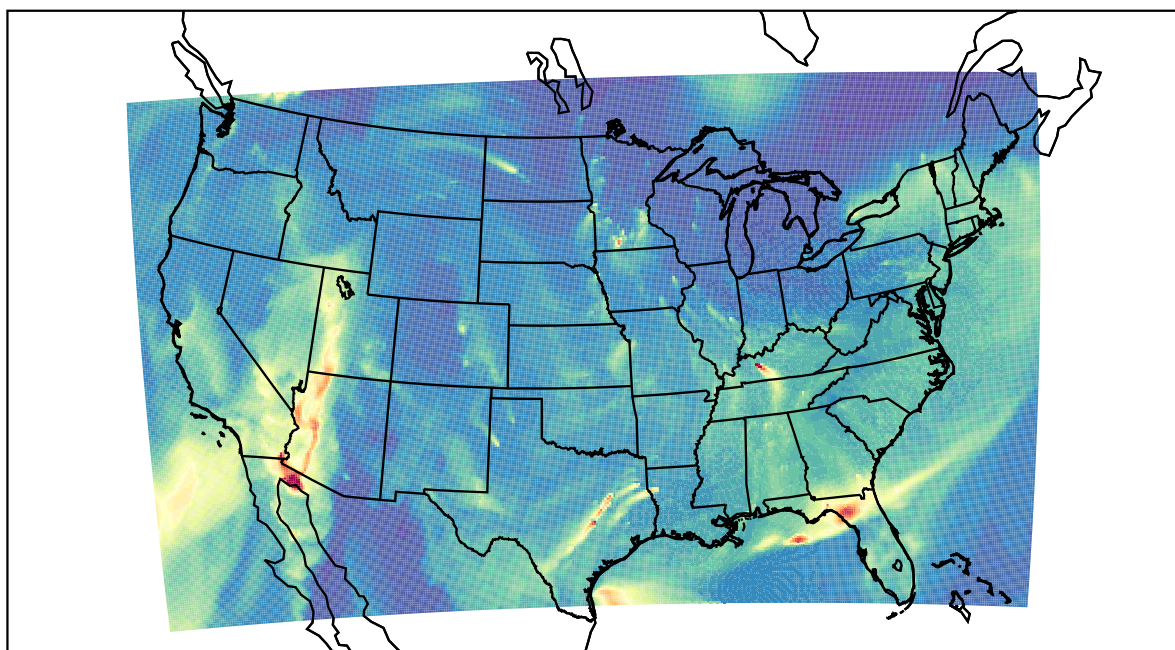
WRF 2019-11-28_10:00:00
