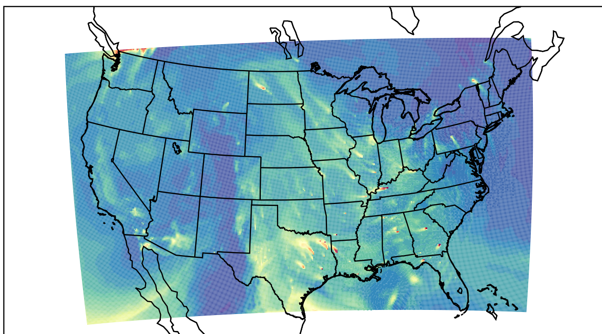
WRF 2019-11-29_19:00:00
