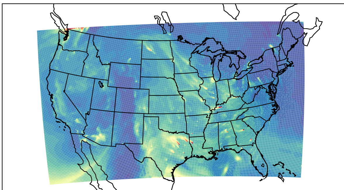
WRF 2019-11-29_18:00:00
