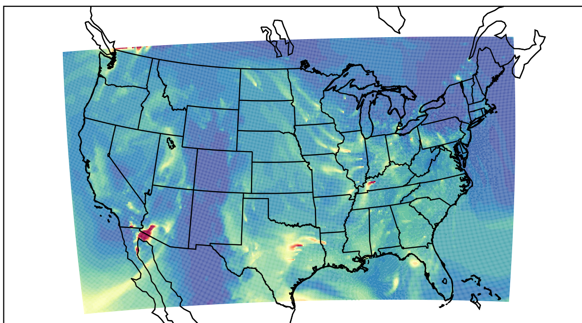
WRF 2019-11-29_12:00:00
