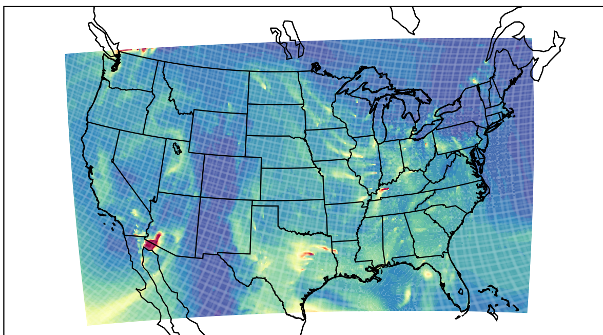
WRF 2019-11-29_13:00:00
