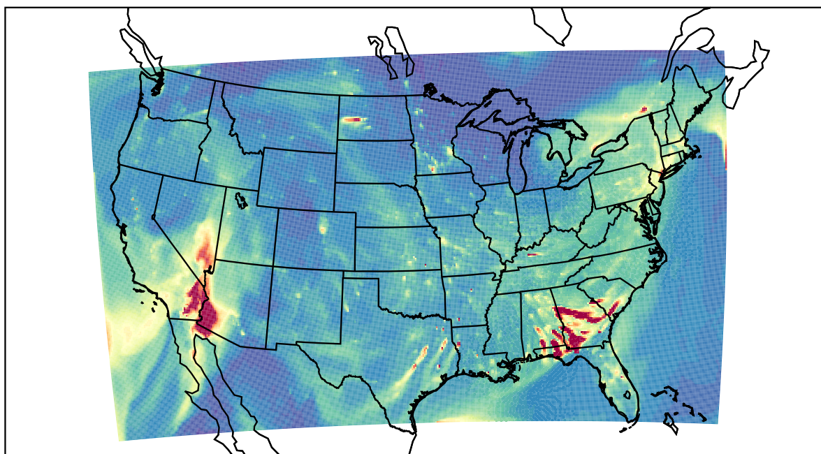
WRF 2019-11-28_01:00:00
