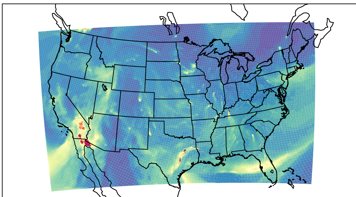
WRF 2019-11-28_17:00:00
