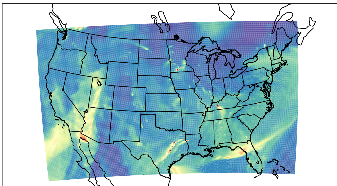
WRF 2019-11-28_12:00:00
