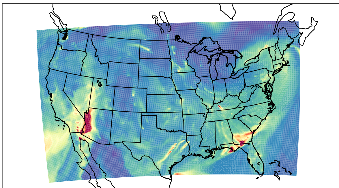
WRF 2019-11-28_06:00:00
