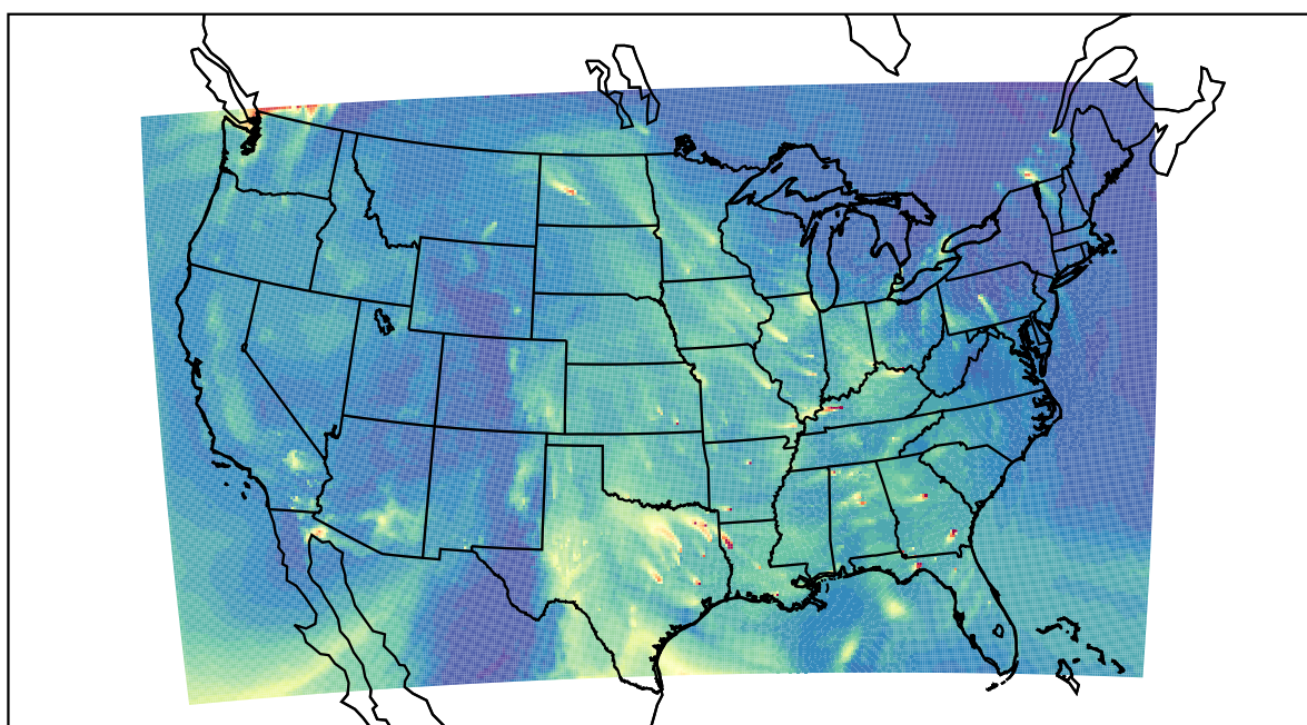
WRF 2019-11-29_20:00:00
