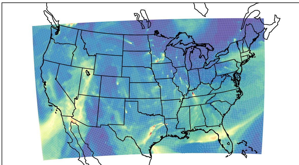
WRF 2019-11-28_14:00:00
