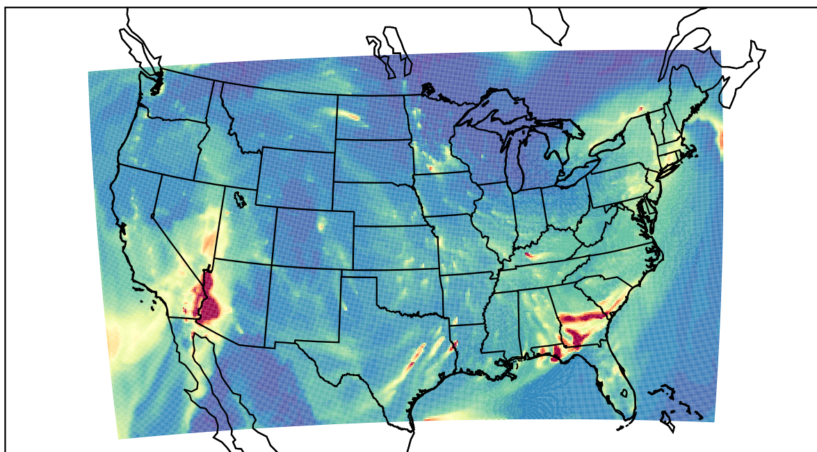
WRF 2019-11-28_04:00:00
