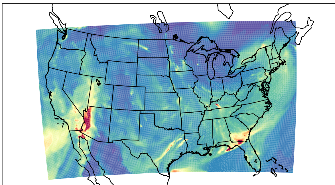
WRF 2019-11-28_07:00:00
