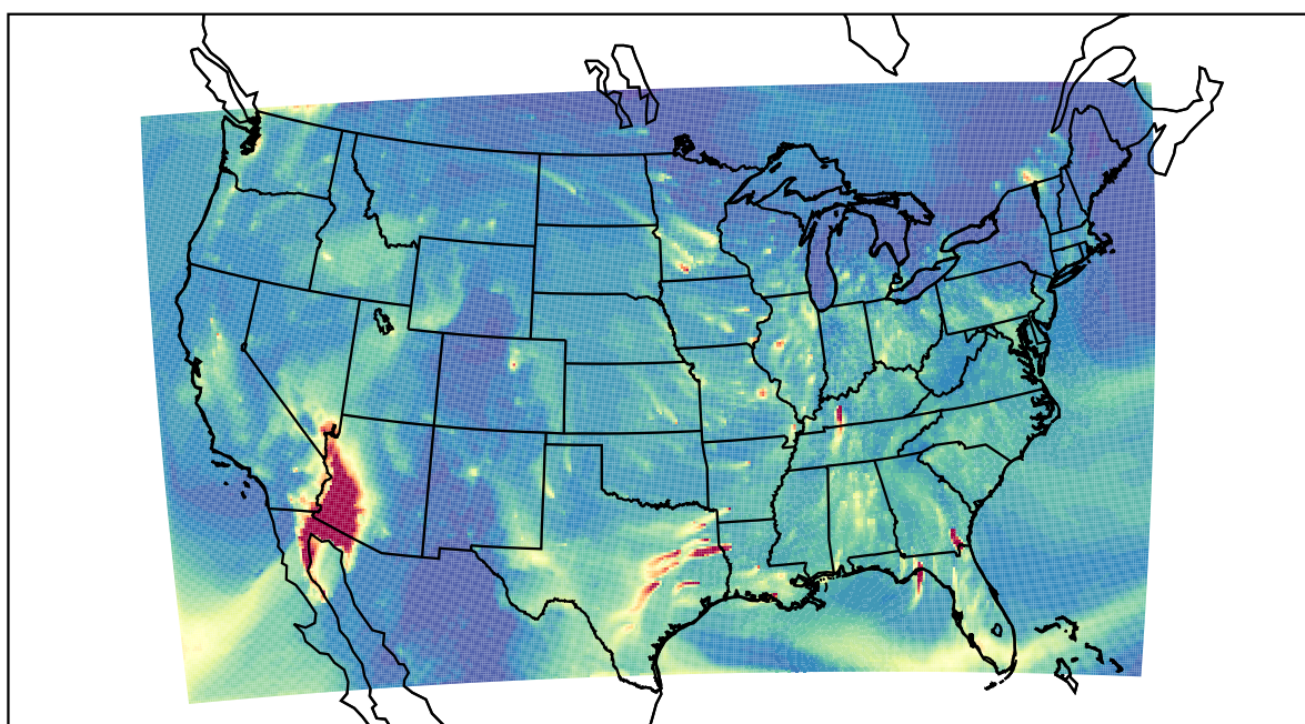
WRF 2019-11-29_02:00:00
