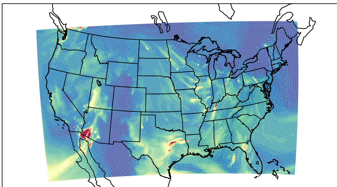
WRF 2019-11-29_08:00:00
