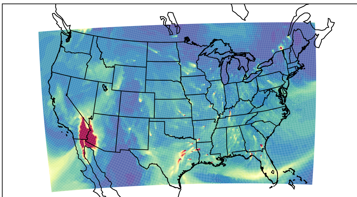
WRF 2019-11-28_22:00:00
