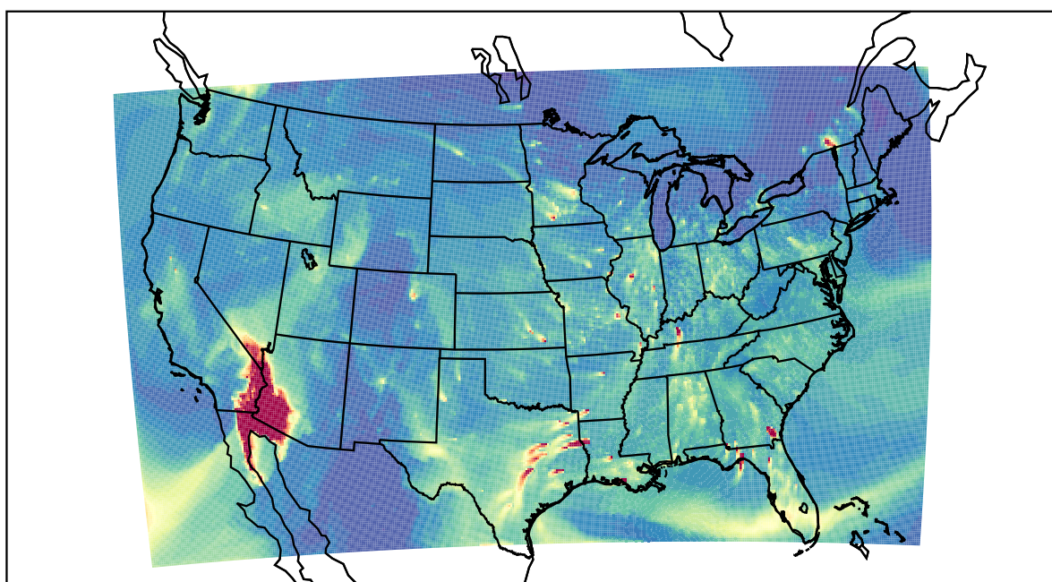
WRF 2019-11-29_00:00:00
