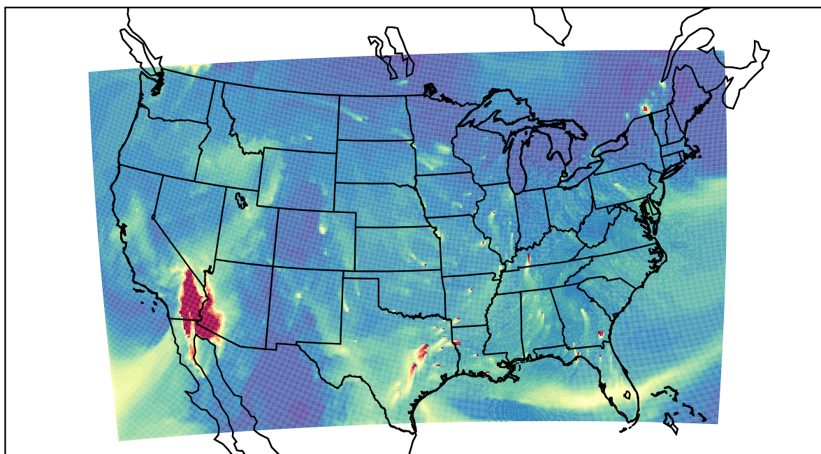
WRF 2019-11-28_21:00:00
