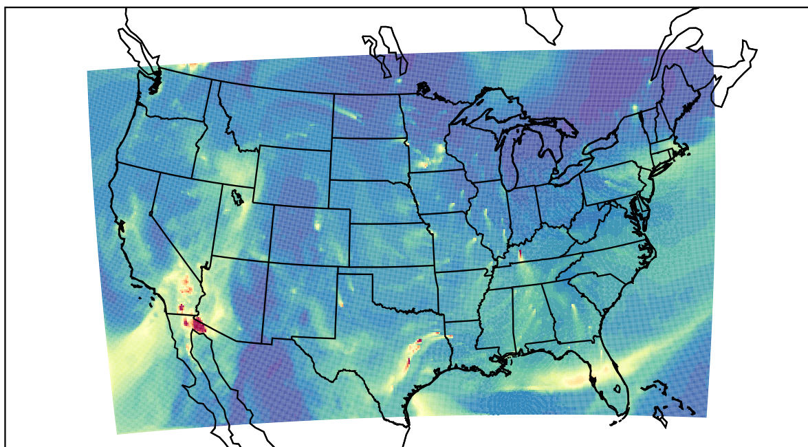
WRF 2019-11-28_16:00:00
