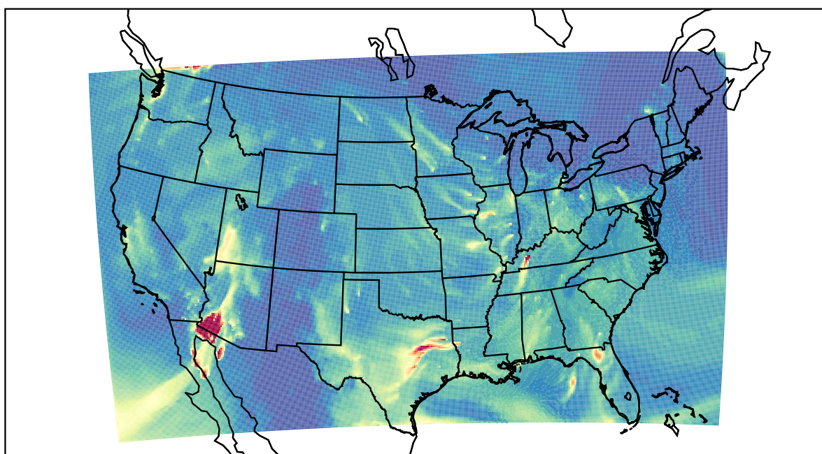
WRF 2019-11-29_07:00:00
