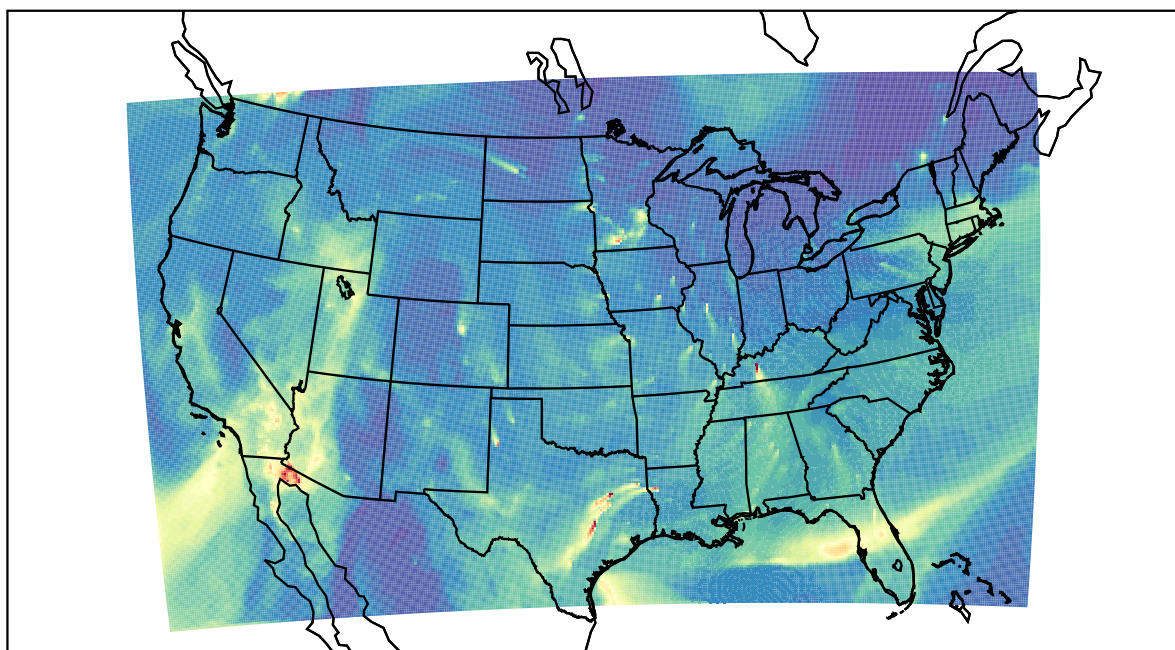
WRF 2019-11-28_15:00:00
