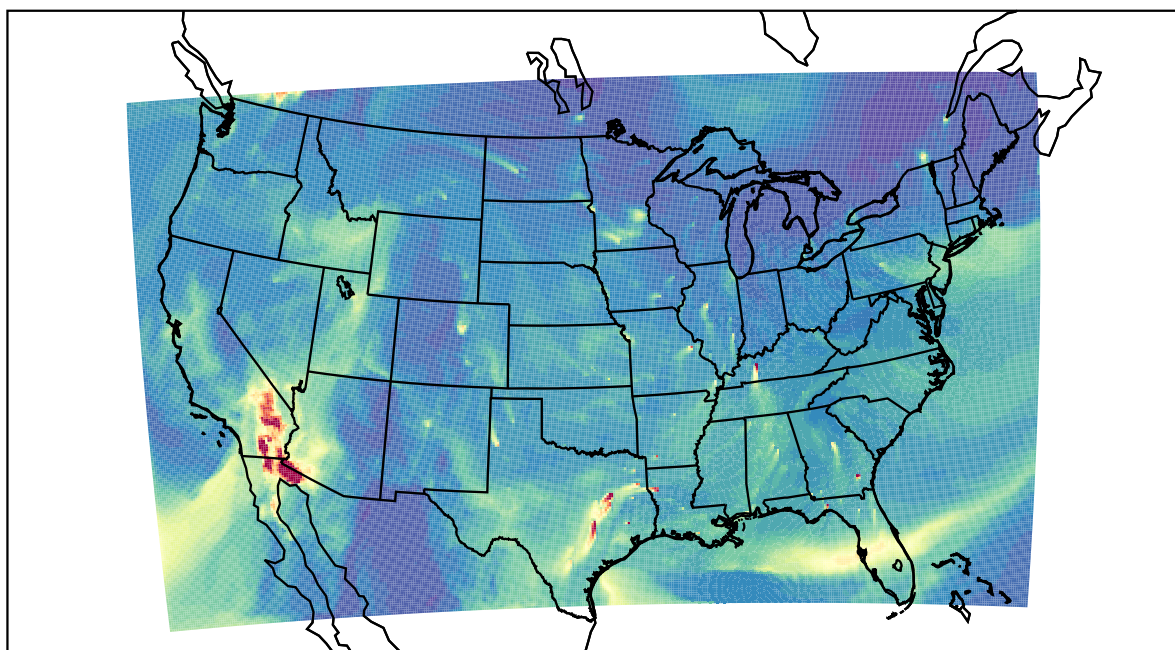
WRF 2019-11-28_18:00:00
