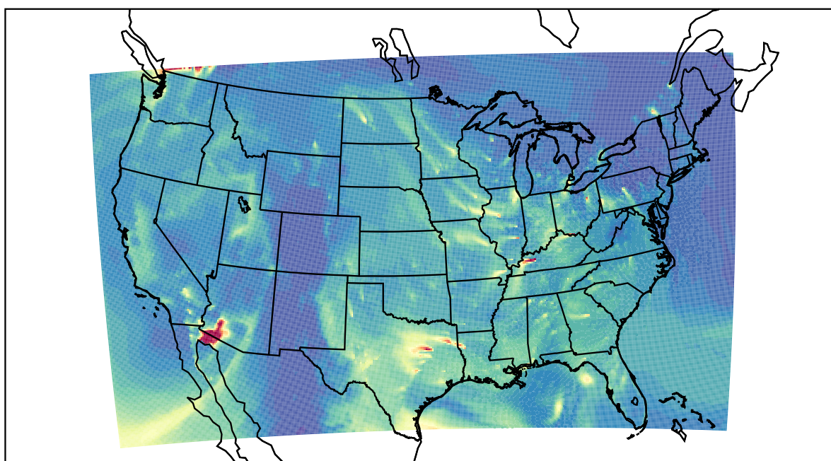
WRF 2019-11-29_14:00:00
