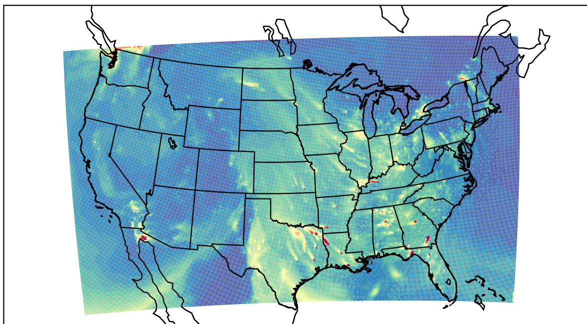
WRF 2019-11-29_23:00:00
