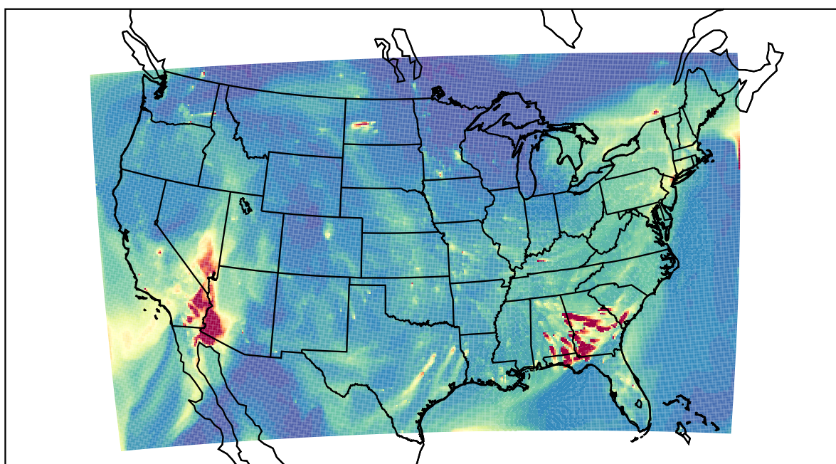
WRF 2019-11-28_00:00:00
