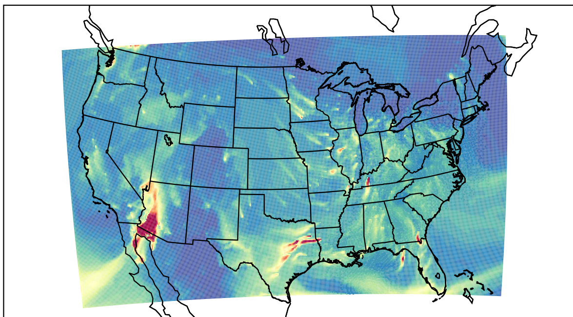
WRF 2019-11-29_04:00:00
