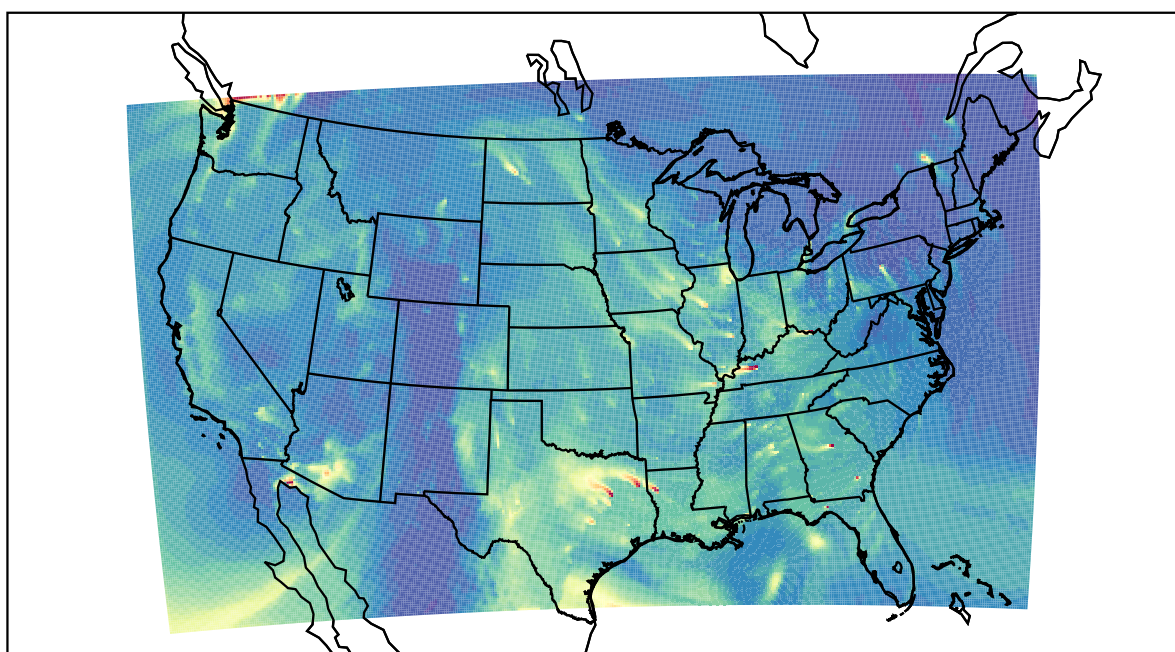
WRF 2019-11-29_17:00:00
