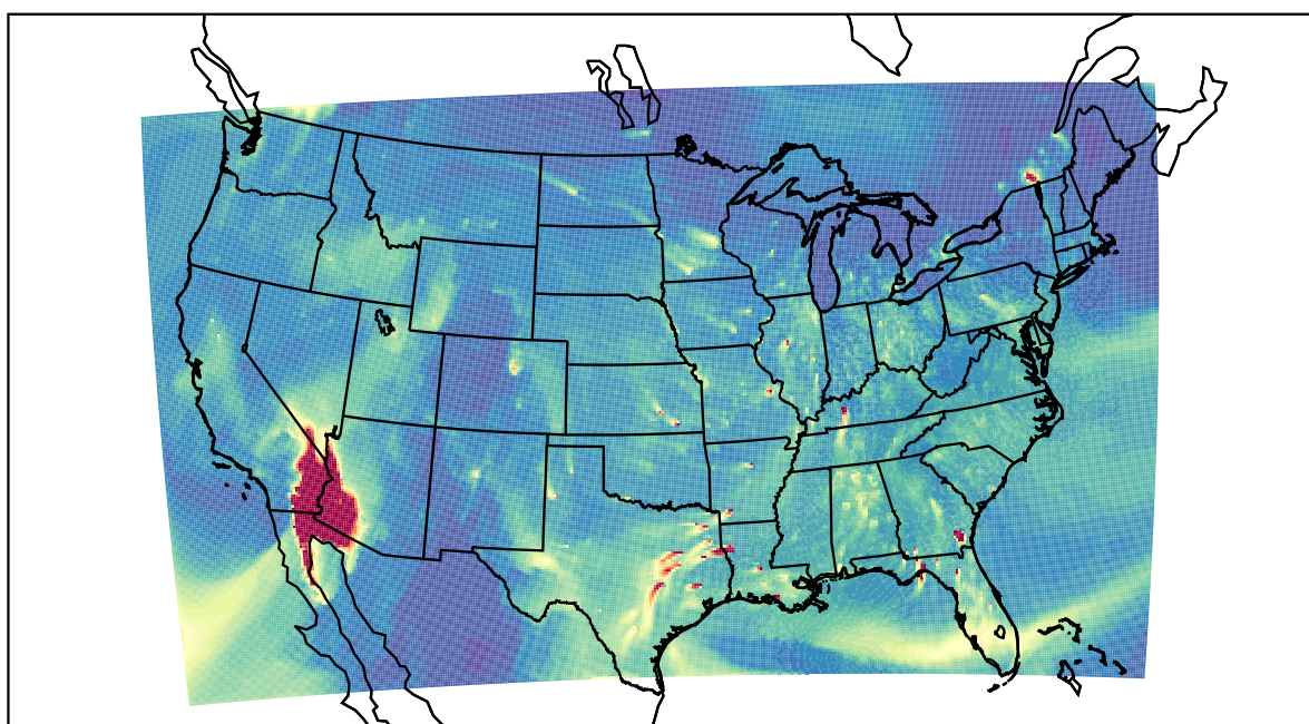
WRF 2019-11-28_23:00:00
