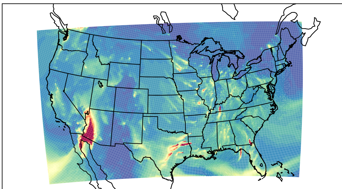
WRF 2019-11-29_03:00:00
