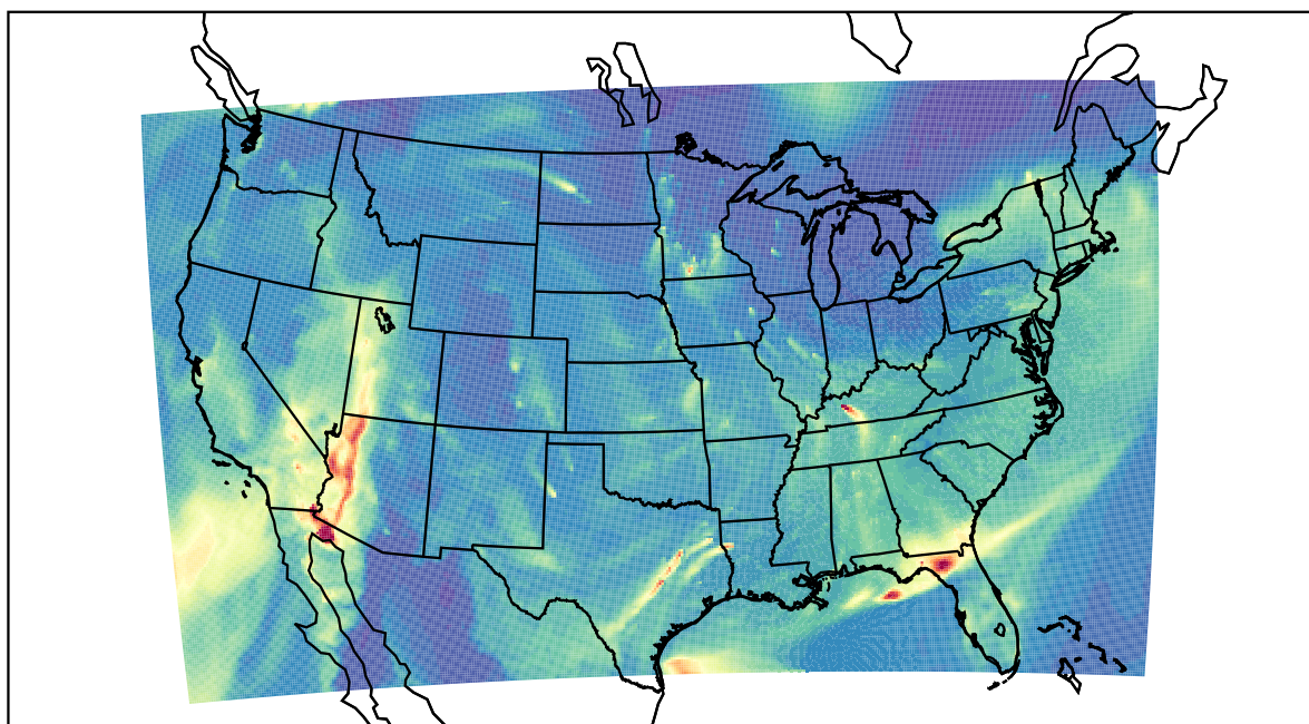
WRF 2019-11-28_09:00:00
