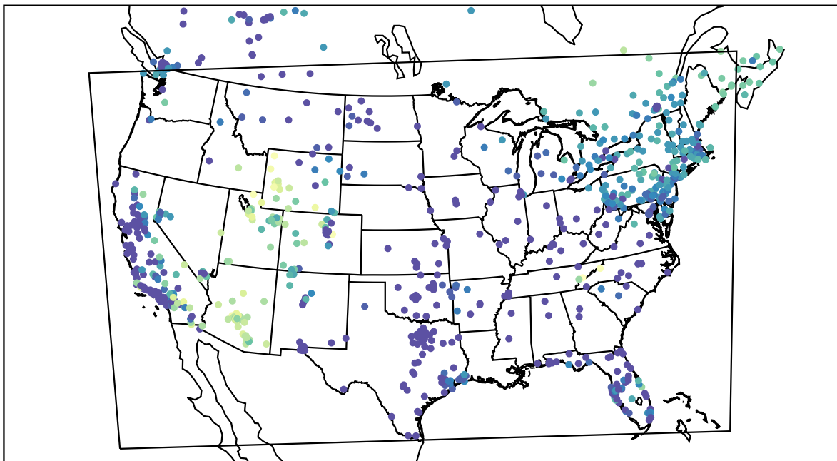
AirNOW (2019-11-29_11:00:00)
