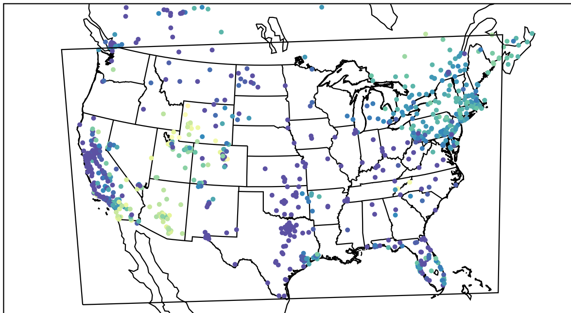
AirNOW (2019-11-29_08:00:00)
