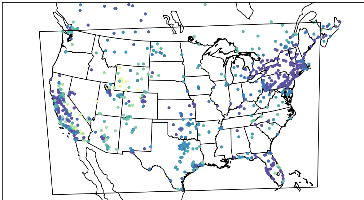
AirNOW (2019-11-28_08:00:00)
