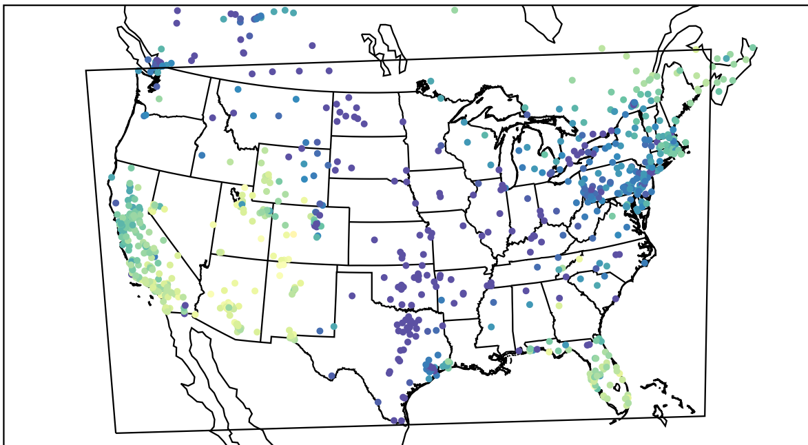
AirNOW (2019-11-29_22:00:00)
