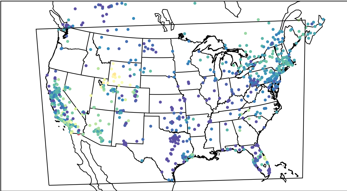
AirNOW (2019-11-29_01:00:00)
