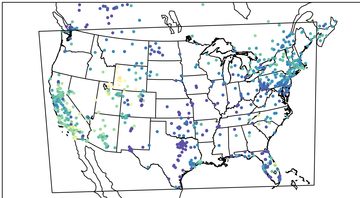
AirNOW (2019-11-29_00:00:00)
