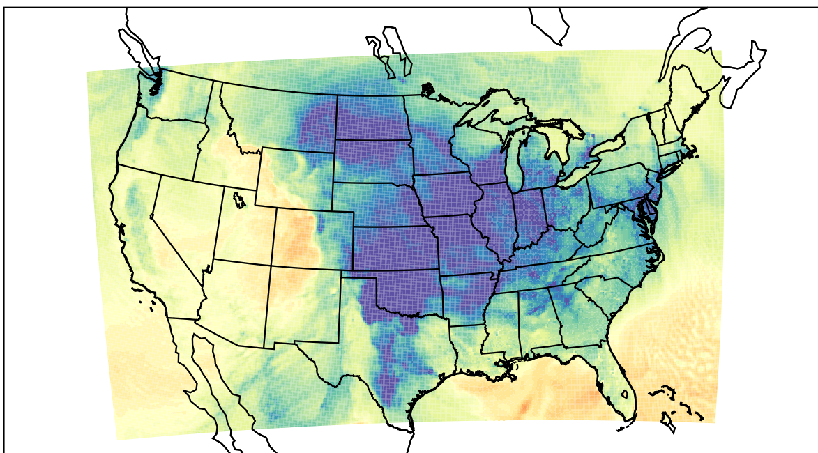
WRF (2019-11-29_22:00:00)
