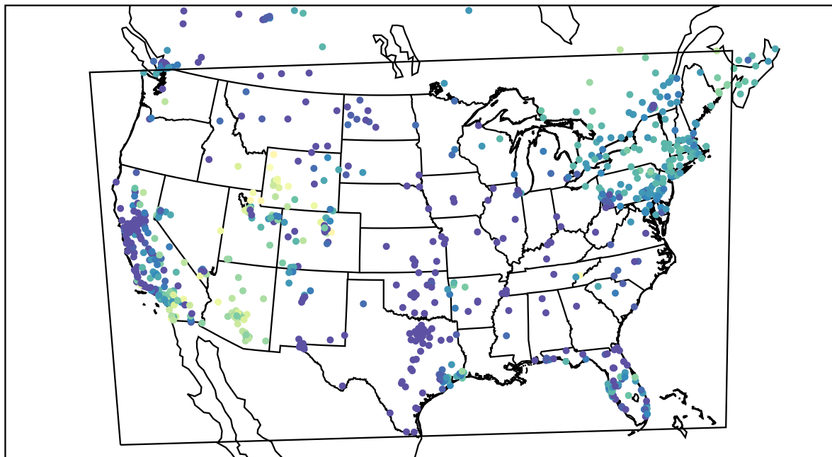
AirNOW (2019-11-29_07:00:00)
