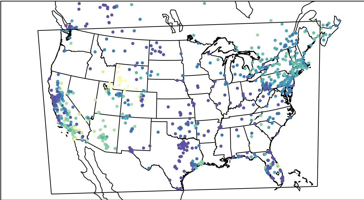
AirNOW (2019-11-29_03:00:00)
