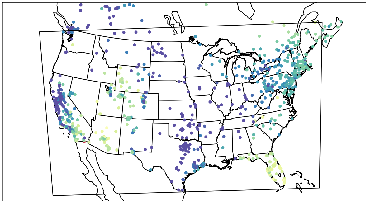
AirNOW (2019-11-29_17:00:00)
