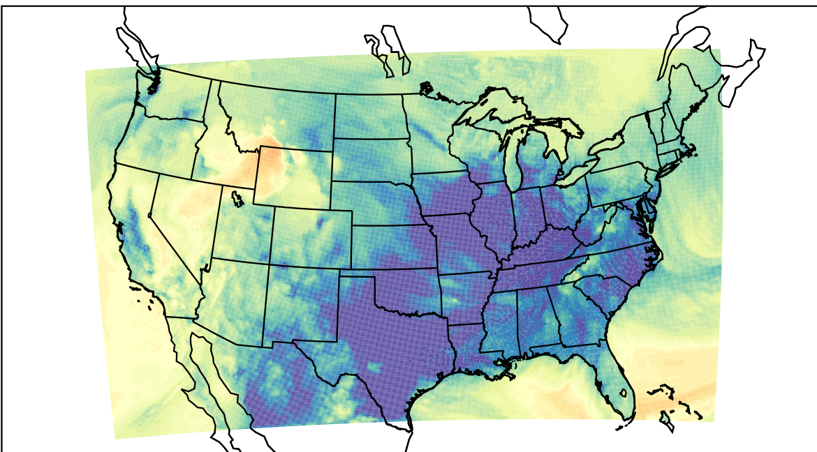
WRF (2019-11-29_06:00:00)
