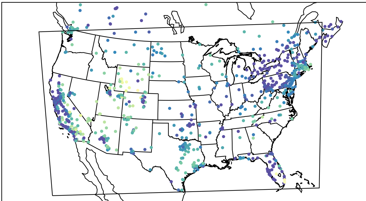
AirNOW (2019-11-28_04:00:00)
