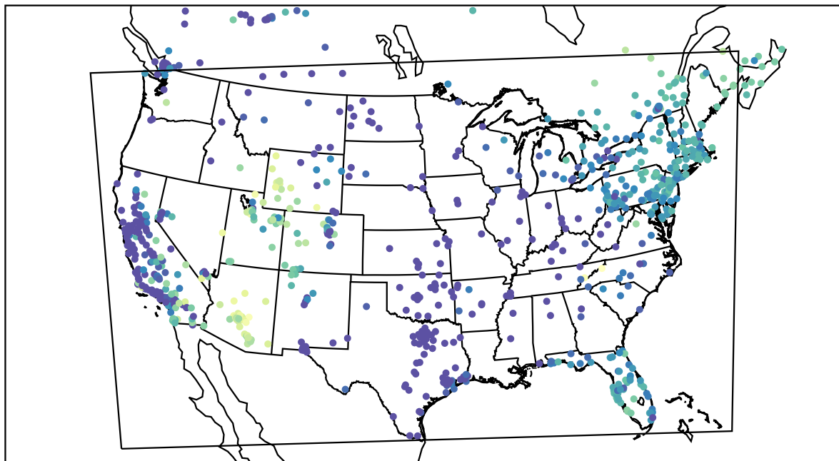
AirNOW (2019-11-29_14:00:00)
