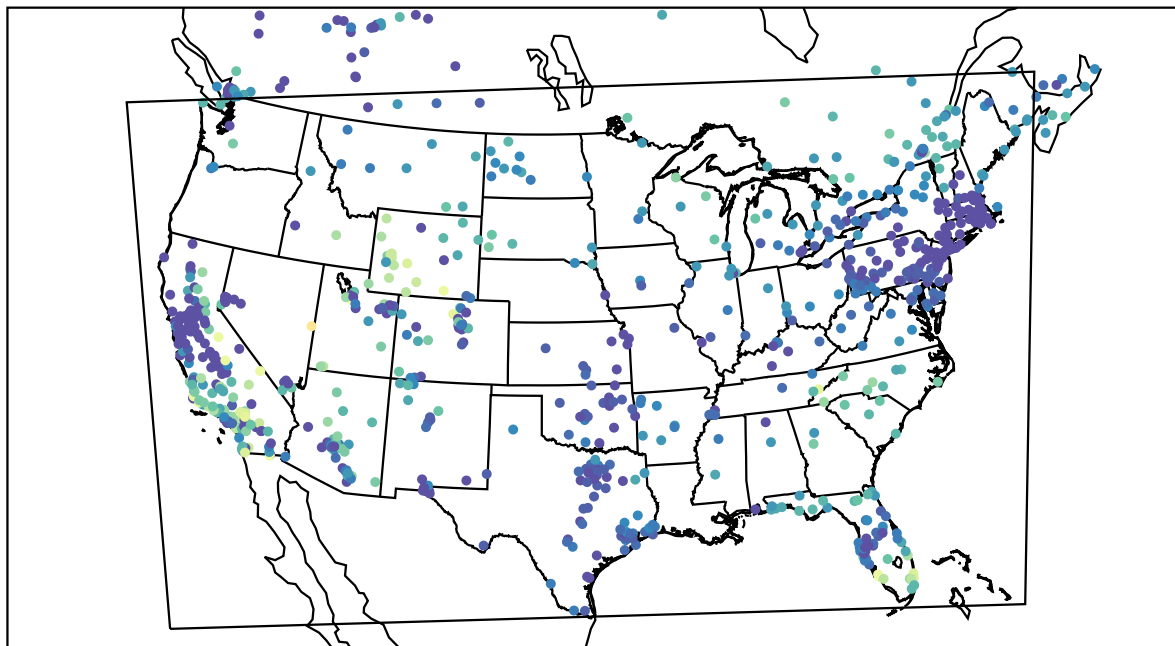
AirNOW (2019-11-28_14:00:00)
