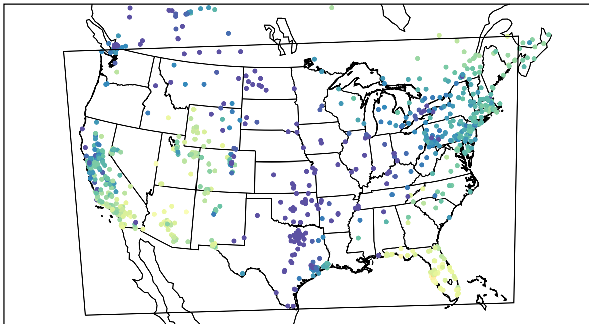
AirNOW (2019-11-29_19:00:00)
