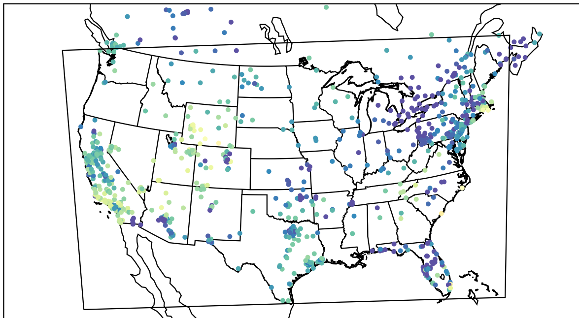
AirNOW (2019-11-28_00:00:00)
