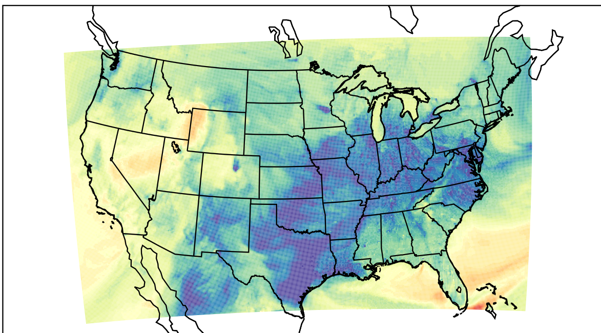
WRF (2019-11-28_23:00:00)
