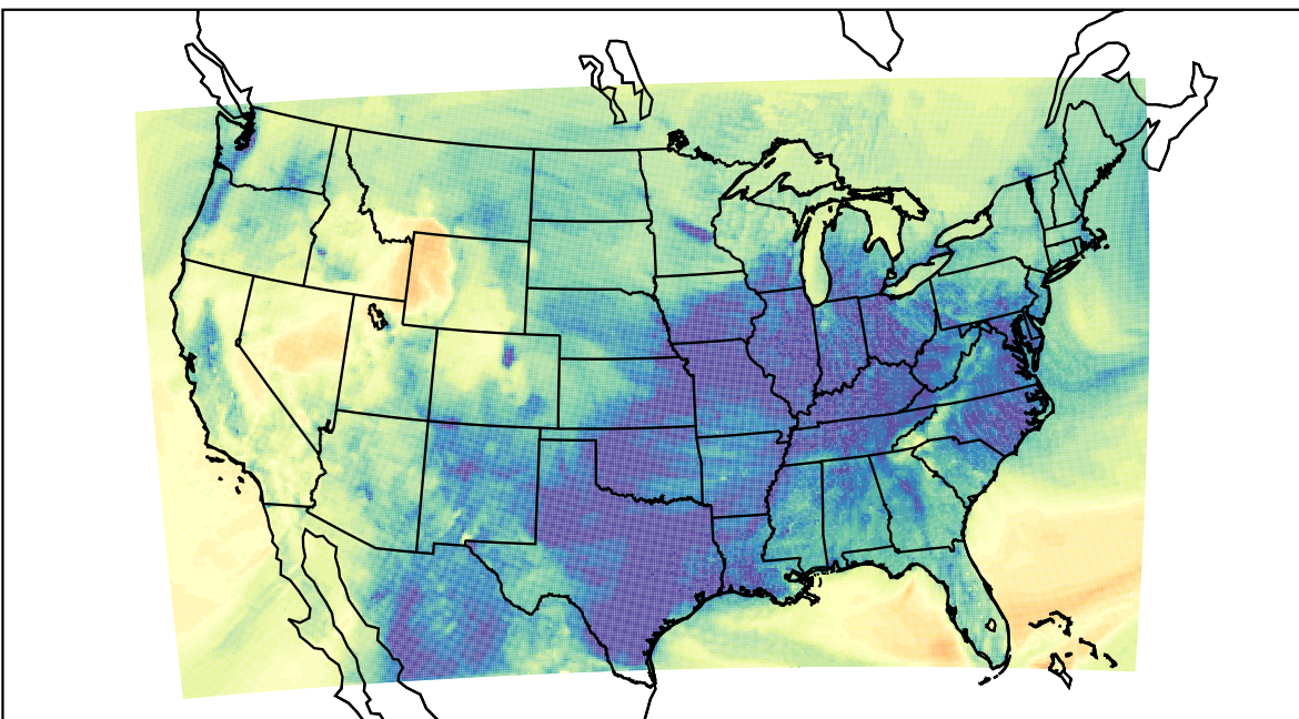
WRF (2019-11-29_01:00:00)
