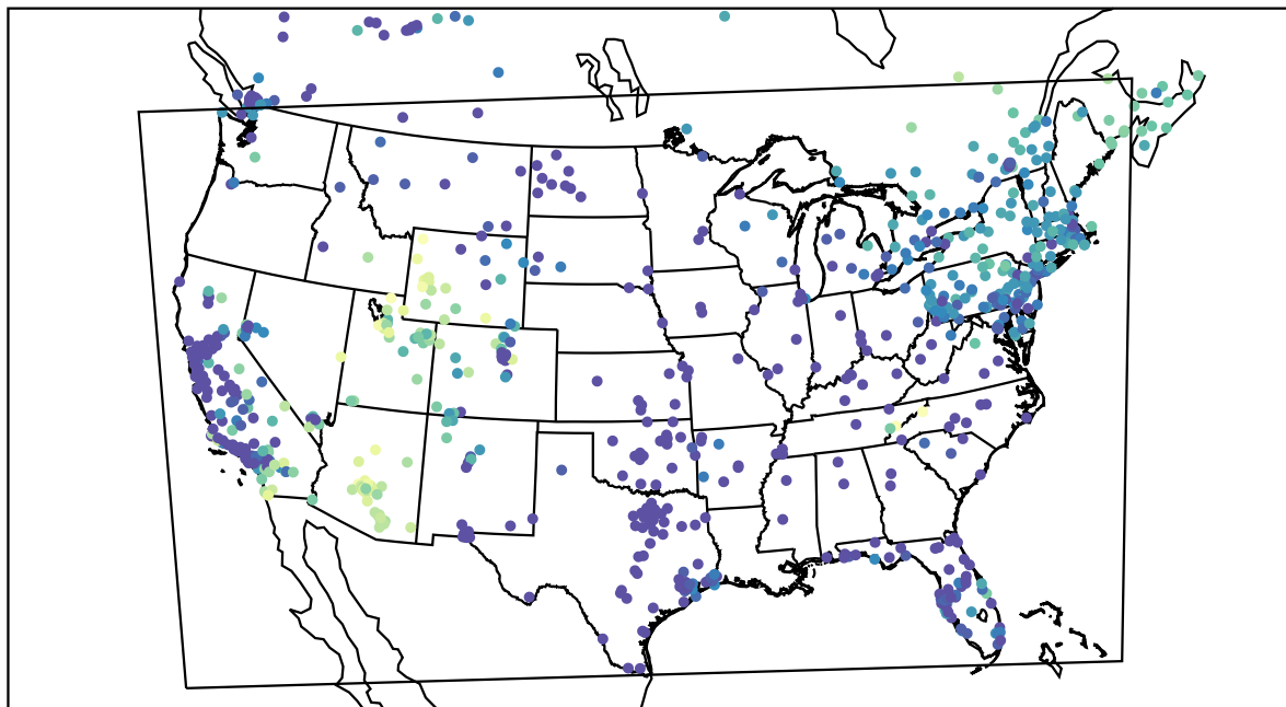
AirNOW (2019-11-29_12:00:00)
