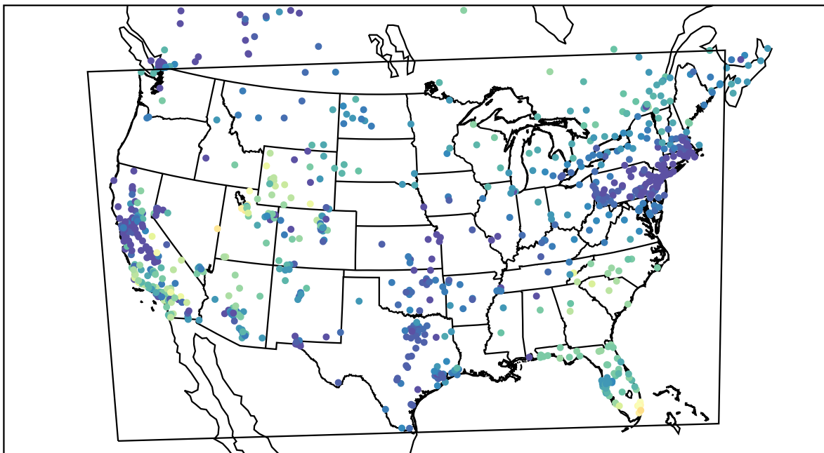
AirNOW (2019-11-28_16:00:00)
