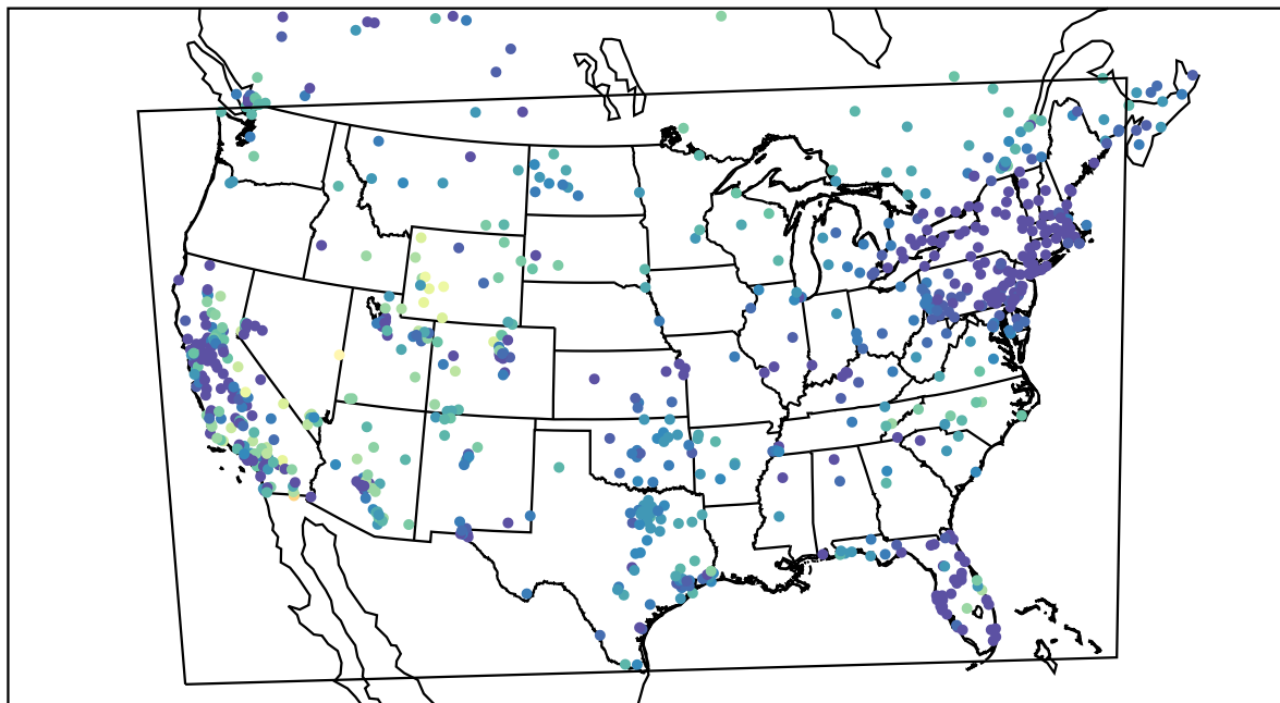
AirNOW (2019-11-28_09:00:00)
