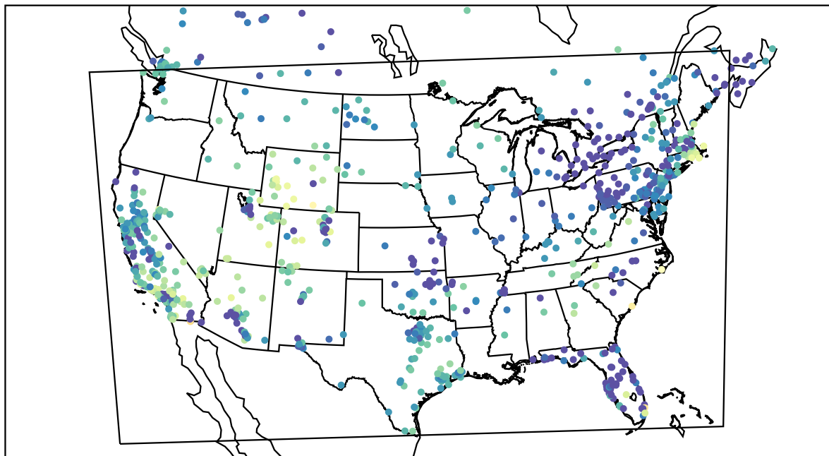
AirNOW (2019-11-28_01:00:00)
