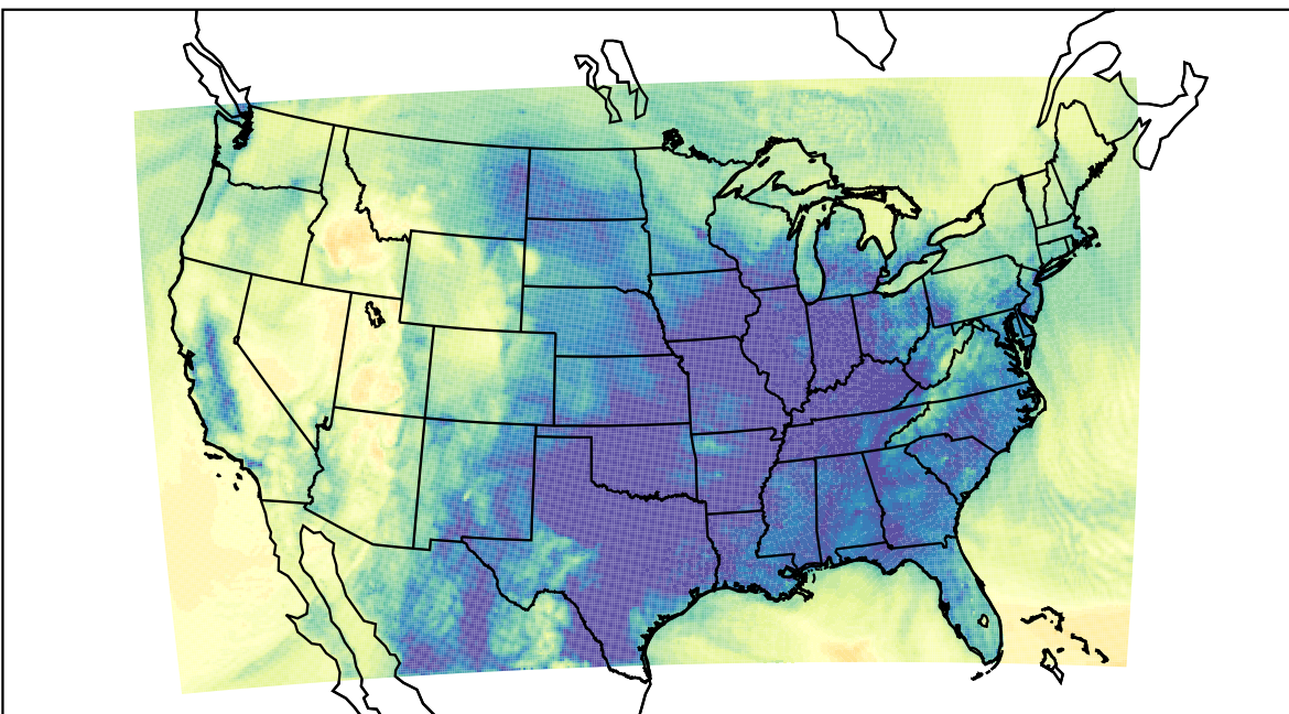
WRF (2019-11-29_13:00:00)
