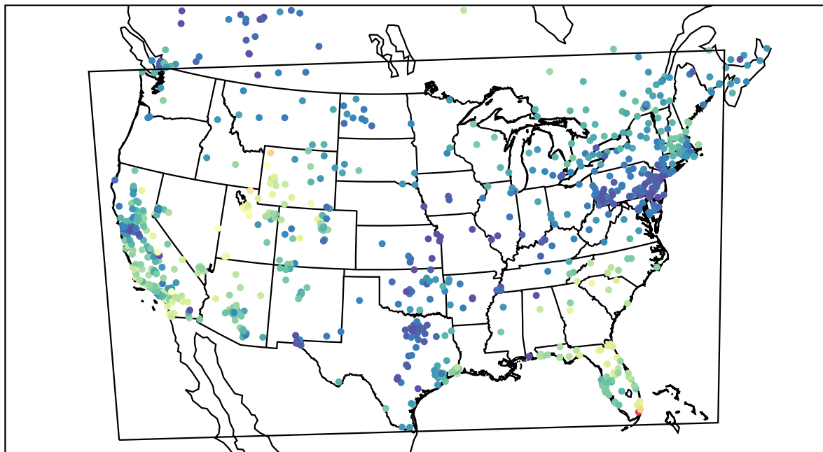
AirNOW (2019-11-28_19:00:00)
