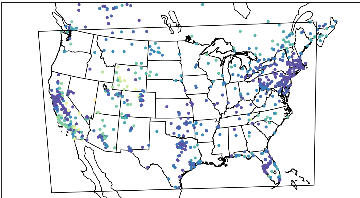
AirNOW (2019-11-28_13:00:00)
