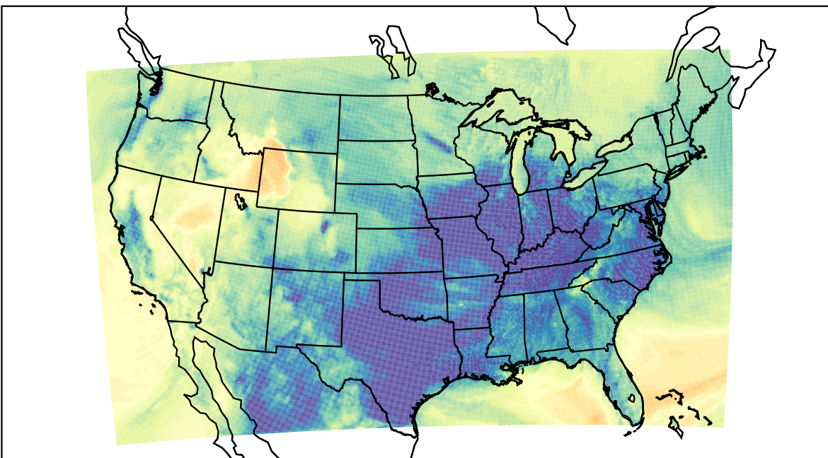
WRF (2019-11-29_03:00:00)
