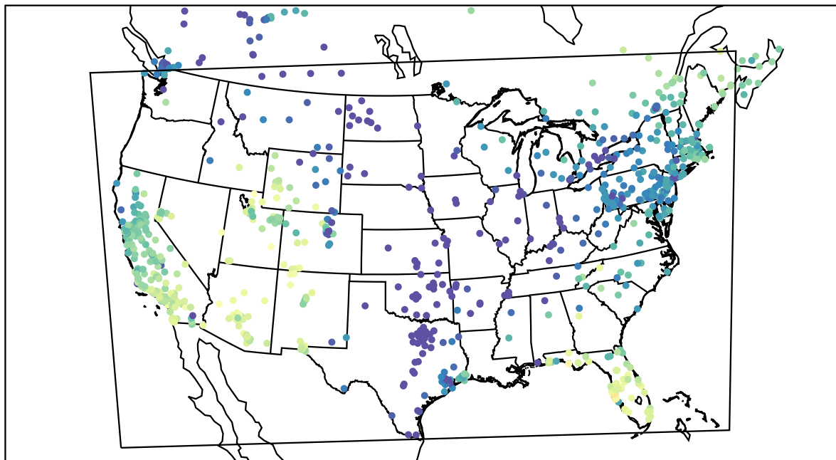
AirNOW (2019-11-29_21:00:00)
