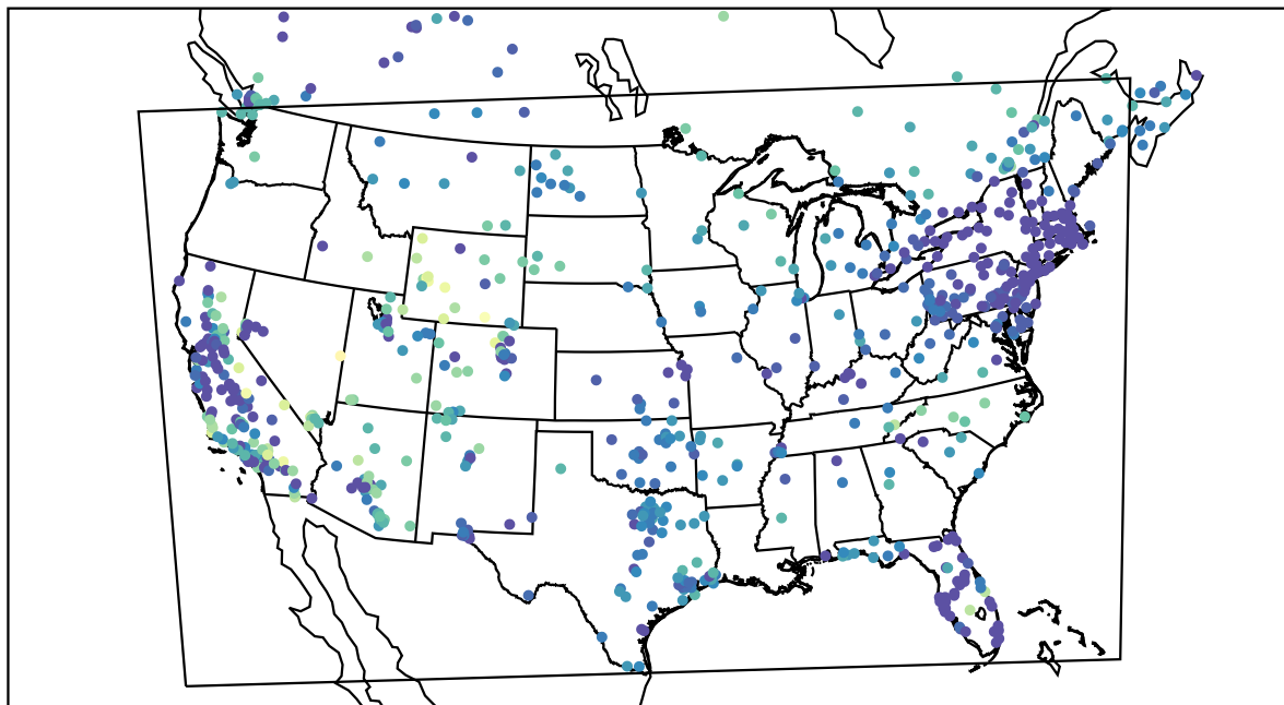
AirNOW (2019-11-28_10:00:00)
