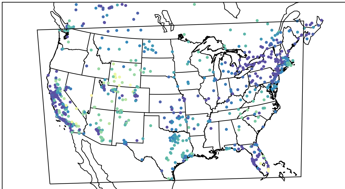
AirNOW (2019-11-28_06:00:00)
