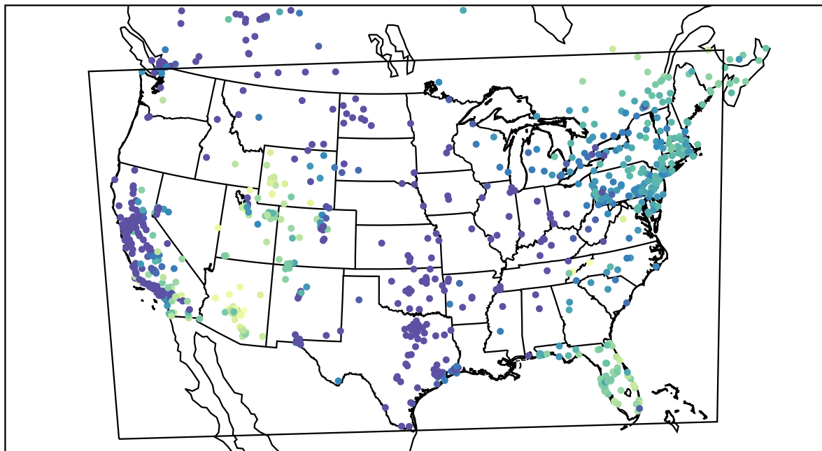
AirNOW (2019-11-29_15:00:00)
