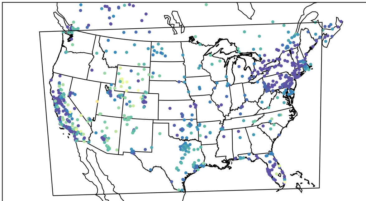
AirNOW (2019-11-28_07:00:00)
