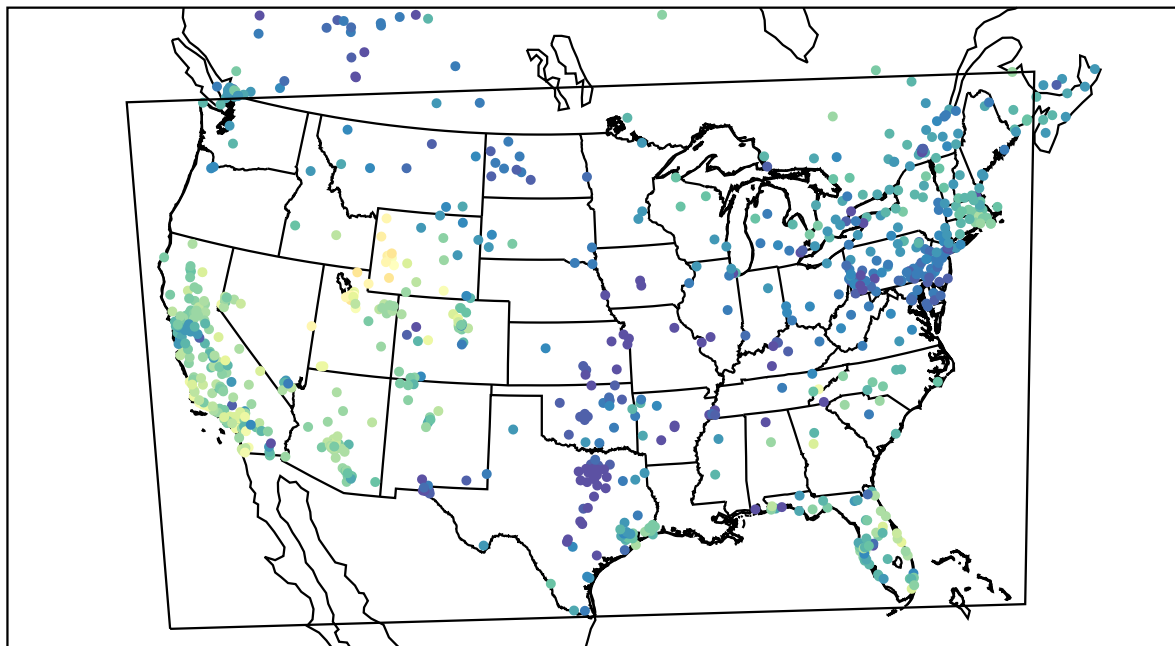
AirNOW (2019-11-28_22:00:00)
