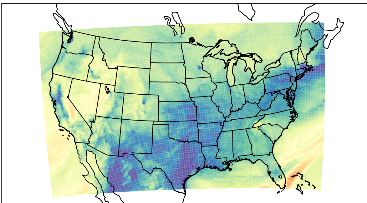
WRF (2019-11-28_16:00:00)
