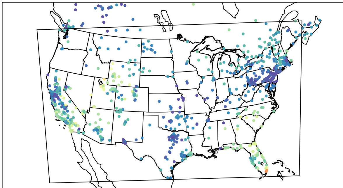
AirNOW (2019-11-28_18:00:00)
