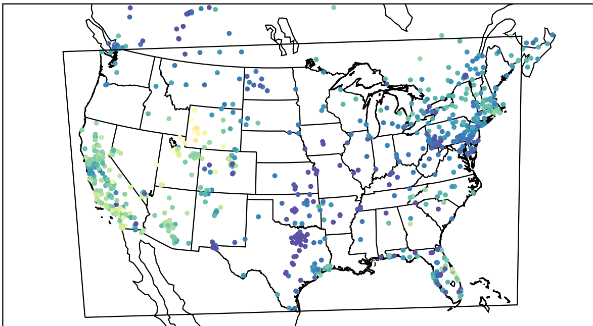
AirNOW (2019-11-28_23:00:00)
