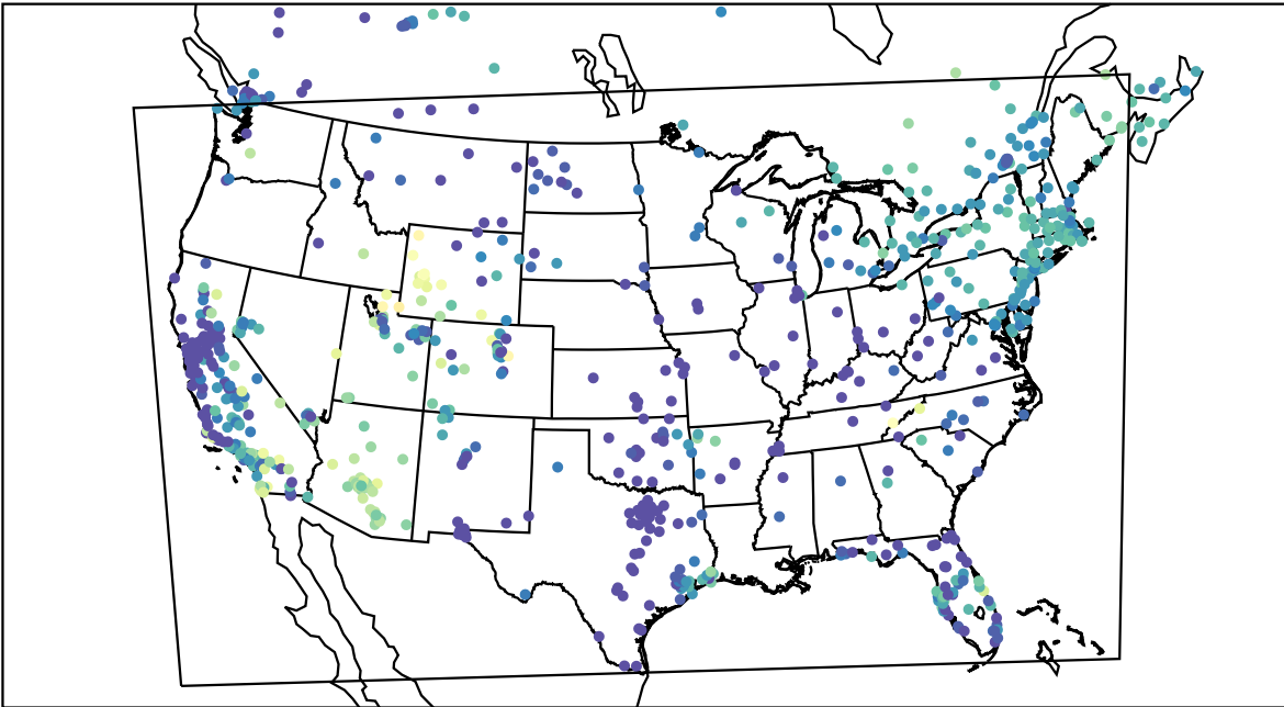
AirNOW (2019-11-29_06:00:00)
