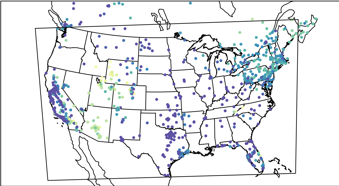
AirNOW (2019-11-29_10:00:00)
