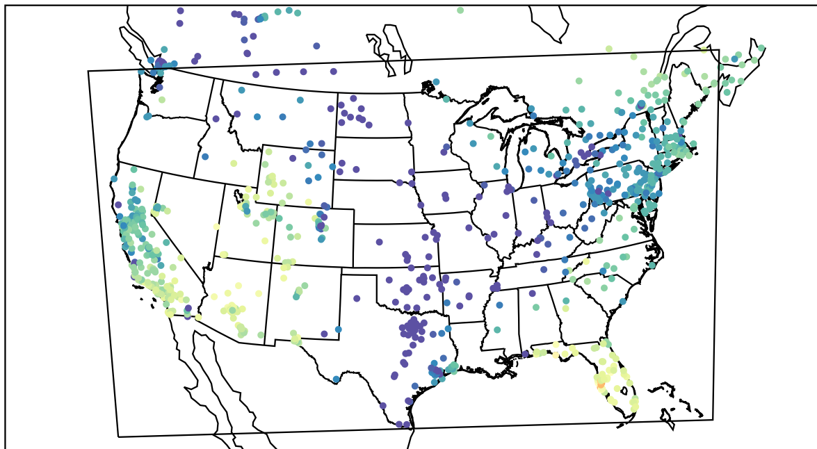
AirNOW (2019-11-29_20:00:00)
