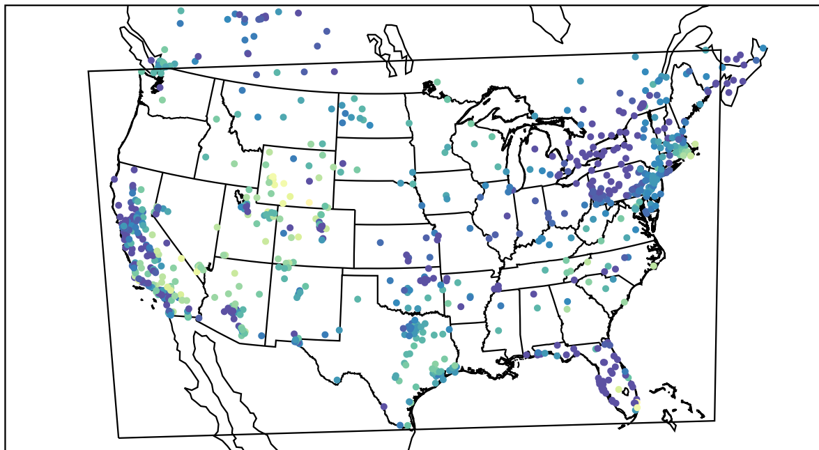
AirNOW (2019-11-28_03:00:00)
