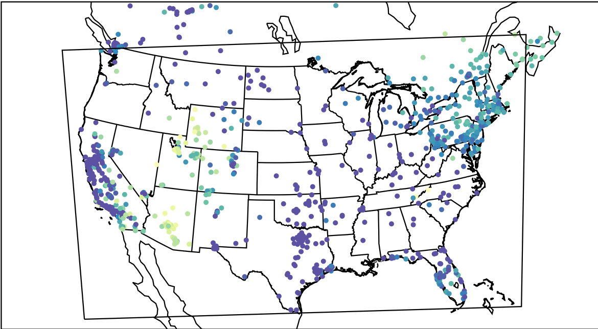
AirNOW (2019-11-29_13:00:00)
