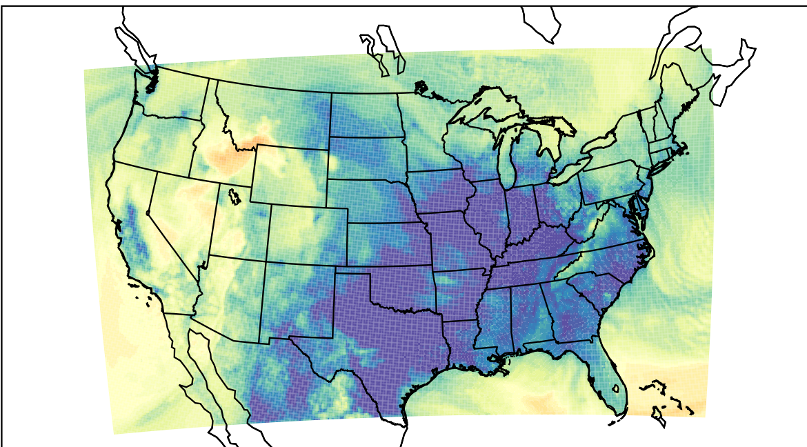
WRF (2019-11-29_10:00:00)
