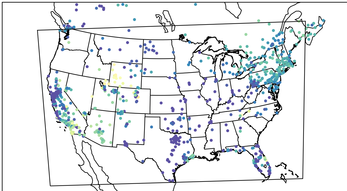
AirNOW (2019-11-29_04:00:00)
