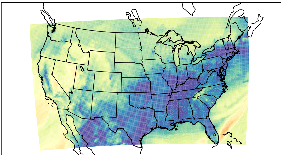
WRF (2019-11-28_13:00:00)
