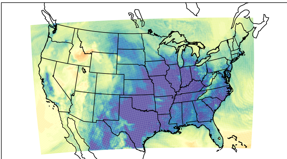
WRF (2019-11-29_11:00:00)
