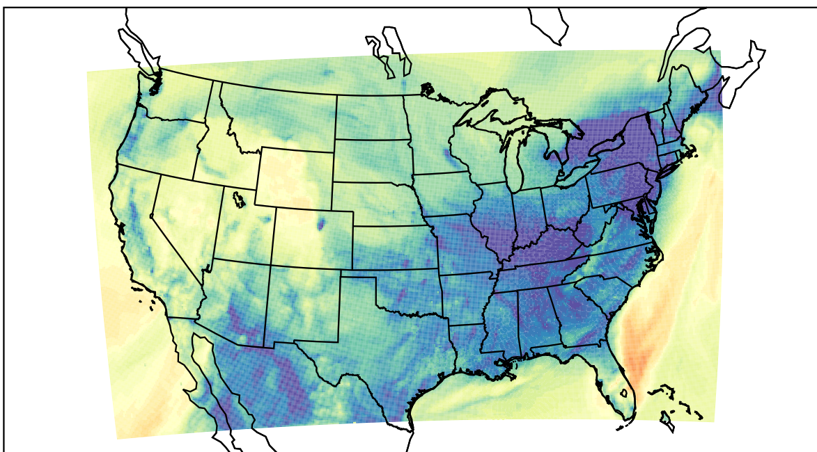
WRF (2019-11-28_04:00:00)
