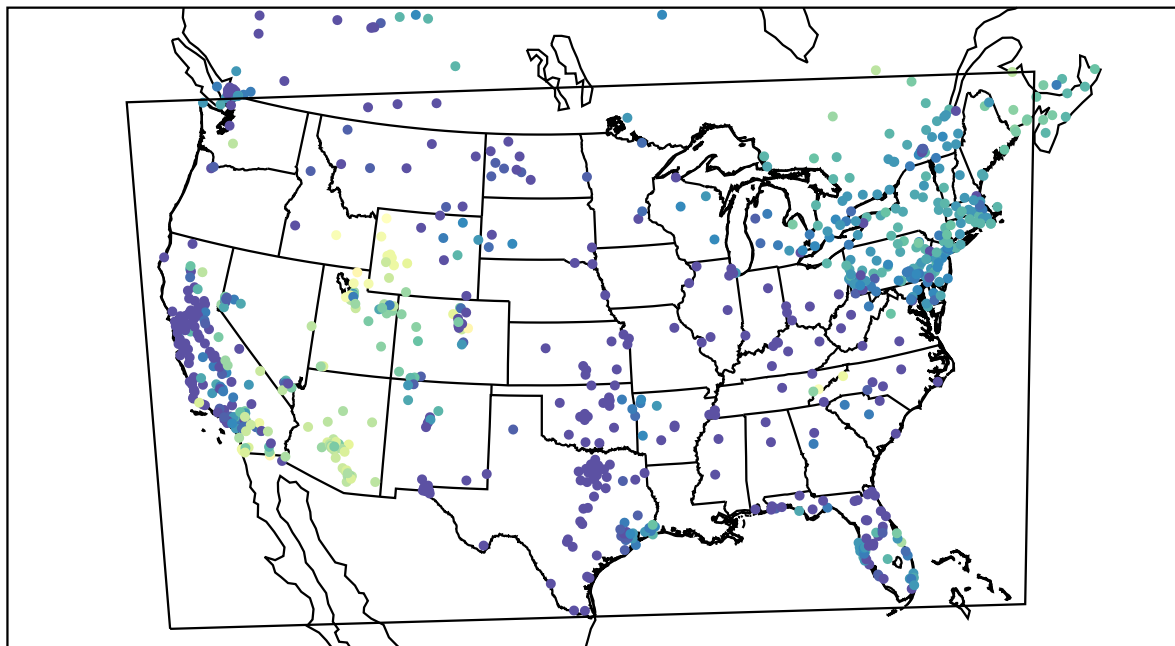
AirNOW (2019-11-29_09:00:00)
