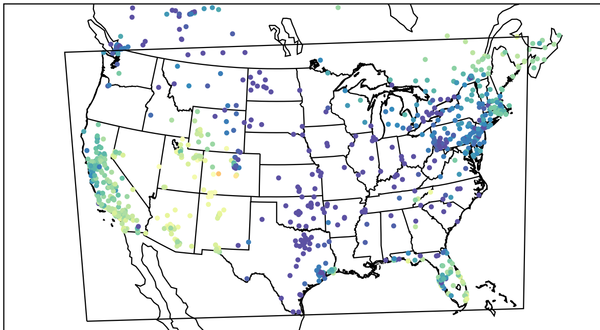
AirNOW (2019-11-29_23:00:00)
