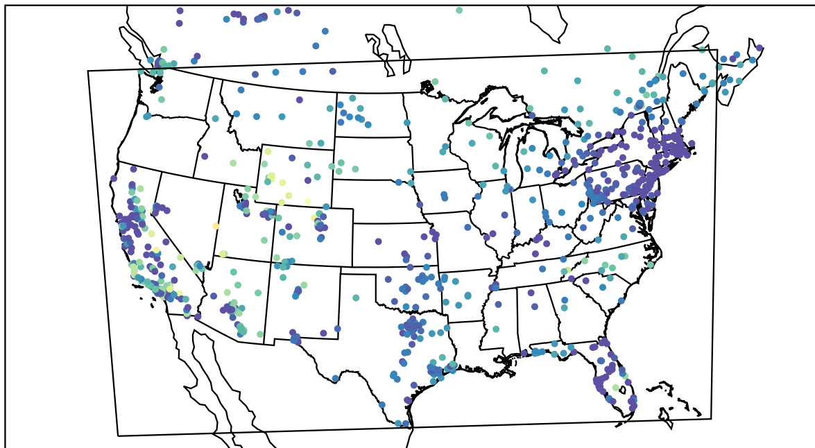
AirNOW (2019-11-28_11:00:00)
