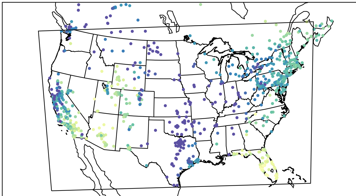
AirNOW (2019-11-29_18:00:00)
