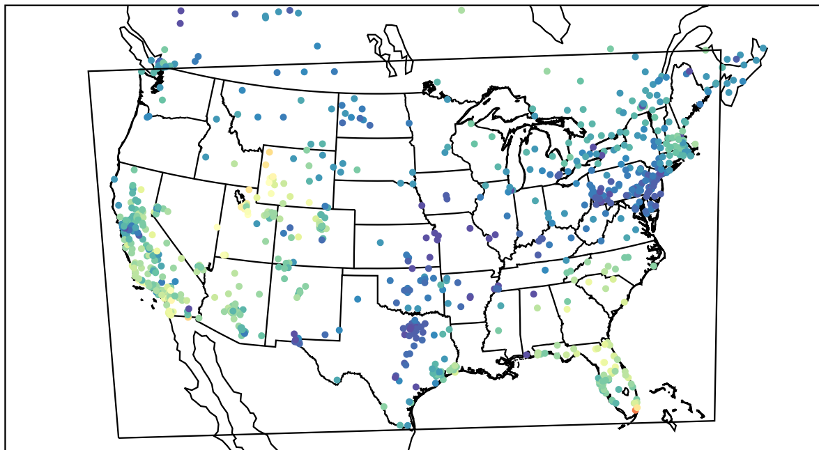
AirNOW (2019-11-28_20:00:00)
