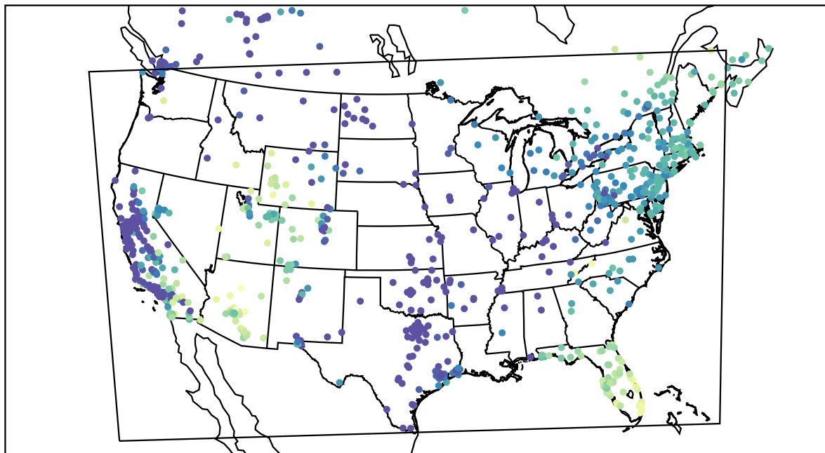
AirNOW (2019-11-29_16:00:00)
