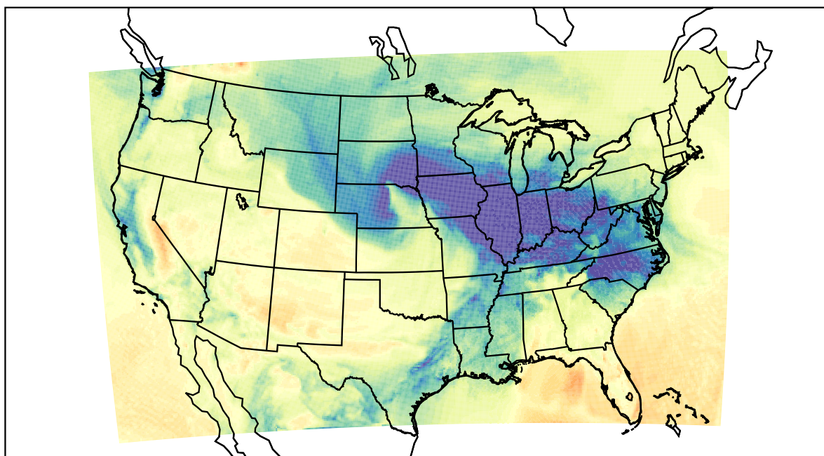
WRF (2019-11-30_18:00:00)
