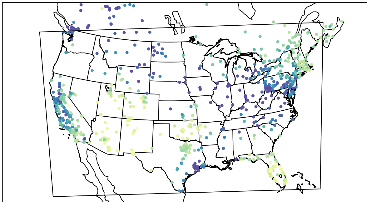
AirNOW (2019-11-30_21:00:00)
