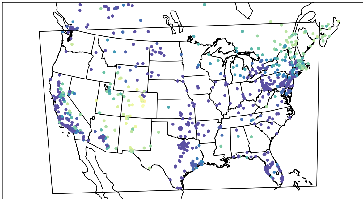
AirNOW (2019-11-30_11:00:00)
