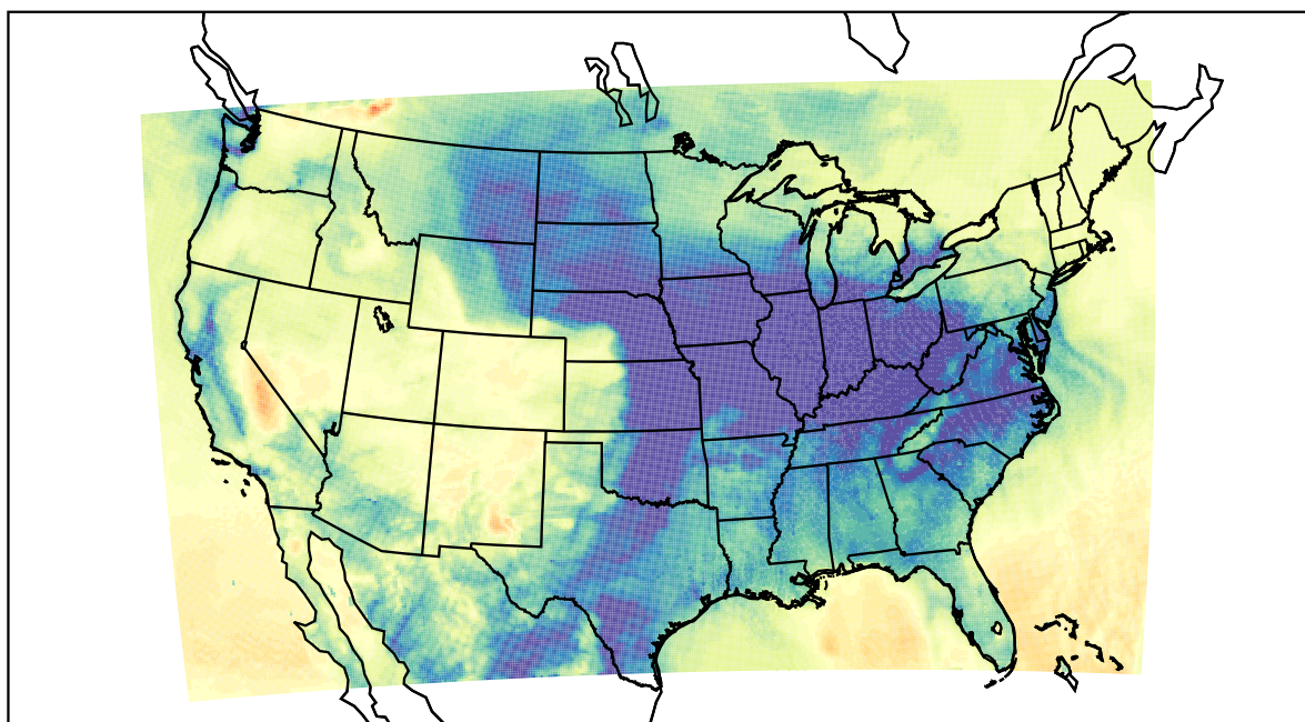
WRF (2019-11-30_10:00:00)
