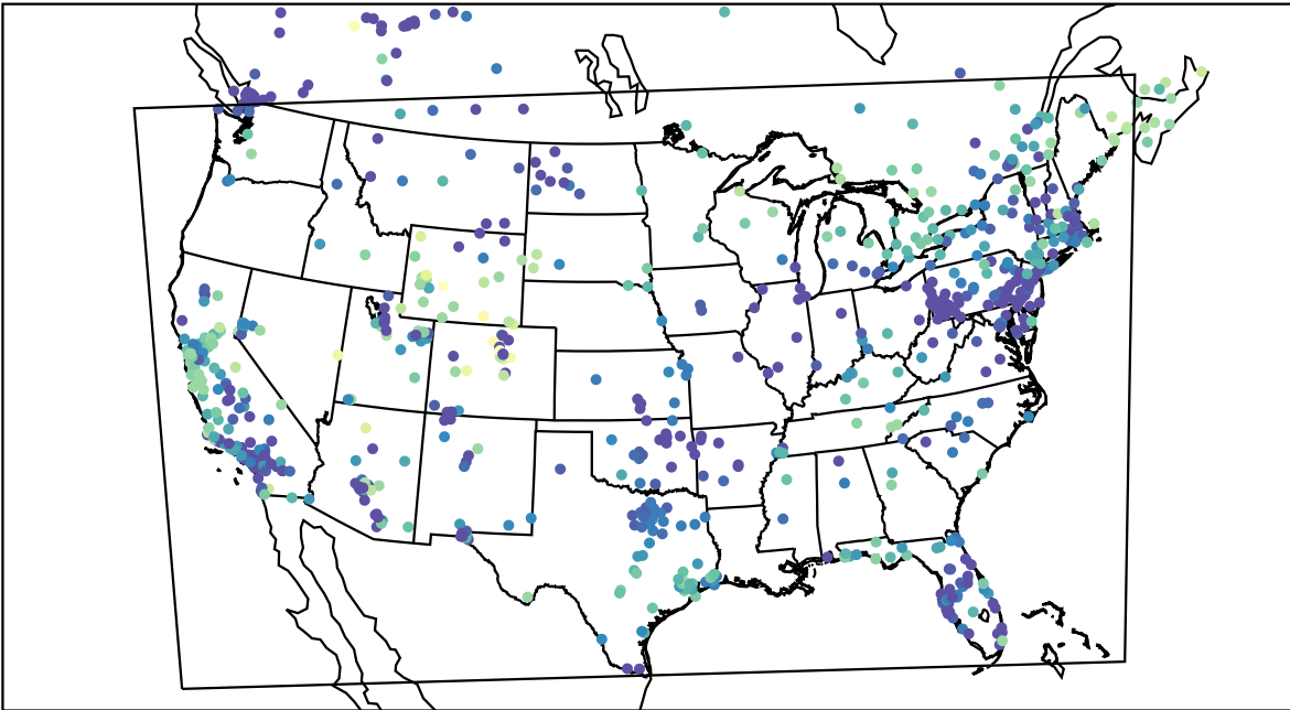
AirNOW (2019-12-01_12:00:00)
