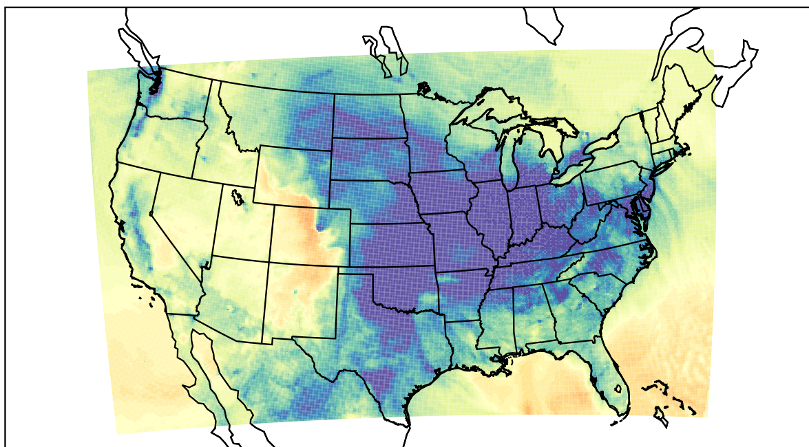
WRF (2019-11-30_02:00:00)
