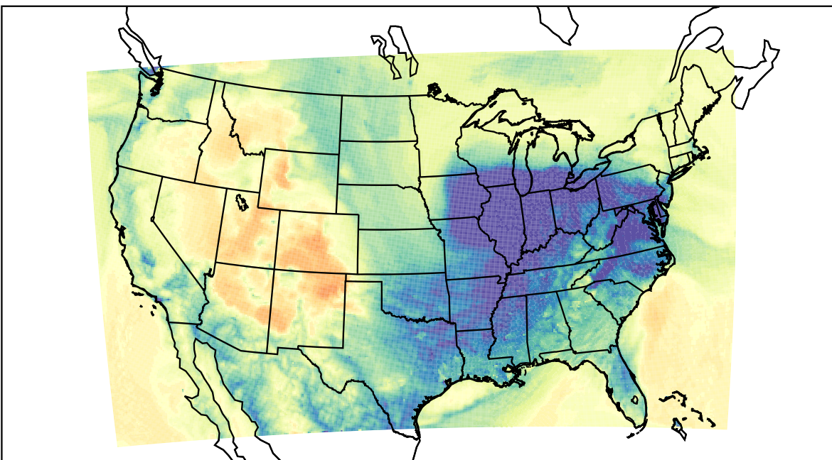
WRF (2019-12-01_12:00:00)
