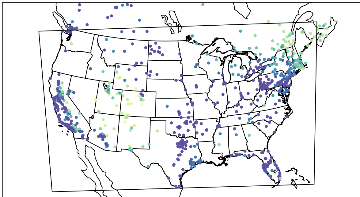
AirNOW (2019-11-30_10:00:00)
