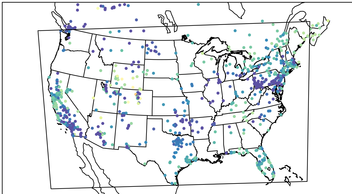
AirNOW (2019-12-01_14:00:00)
