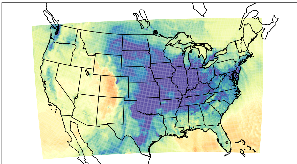
WRF (2019-11-30_00:00:00)
