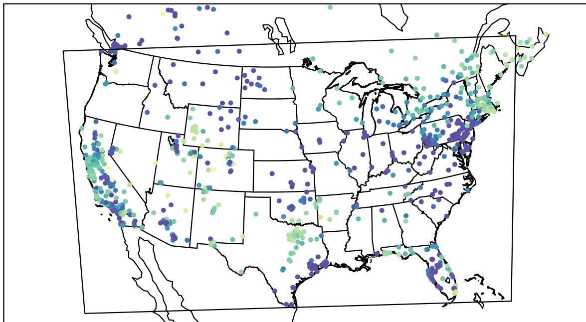
AirNOW (2019-12-01_03:00:00)
