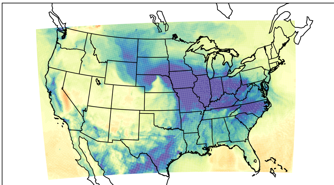
WRF (2019-11-30_15:00:00)
