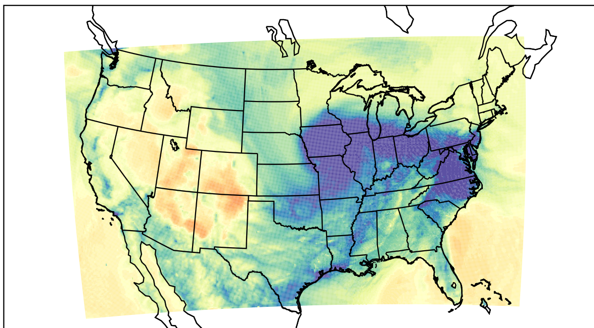
WRF (2019-12-01_07:00:00)
