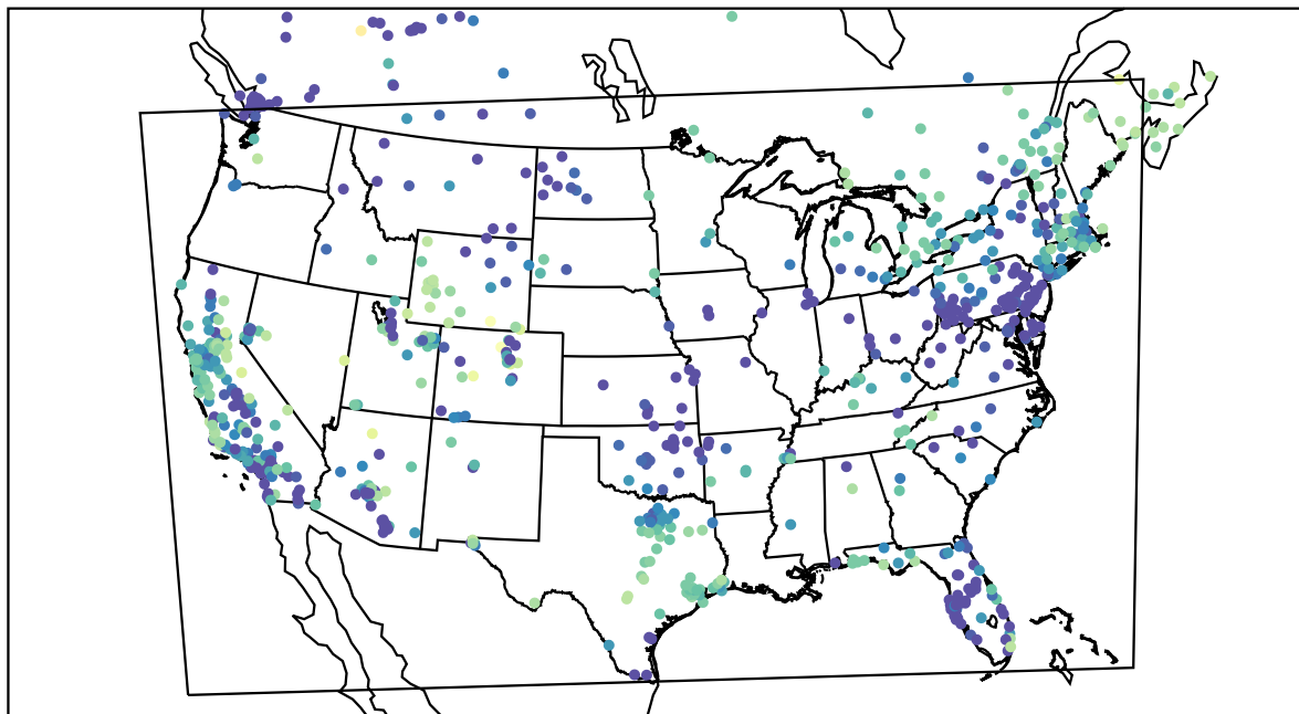
AirNOW (2019-12-01_08:00:00)
