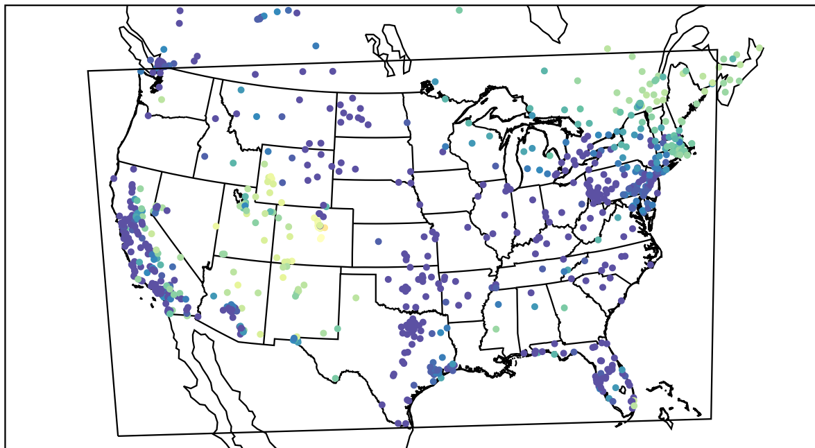
AirNOW (2019-11-30_09:00:00)
