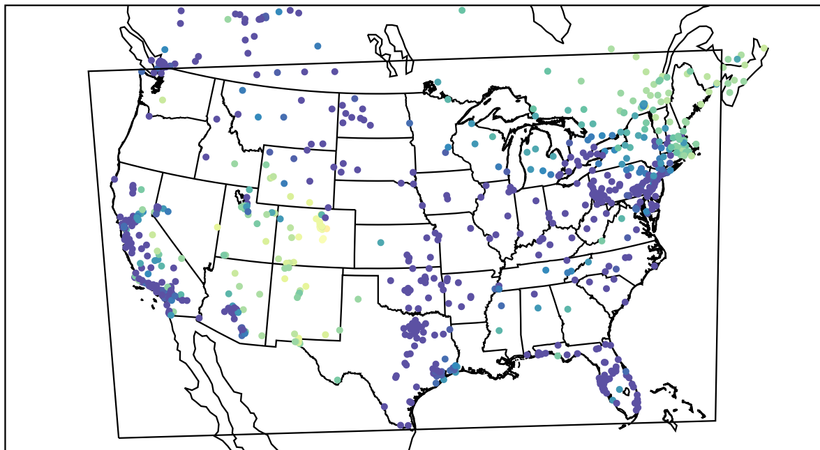
AirNOW (2019-11-30_12:00:00)
