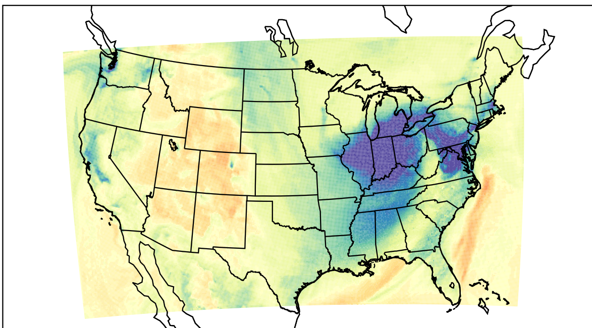
WRF (2019-12-01_21:00:00)
