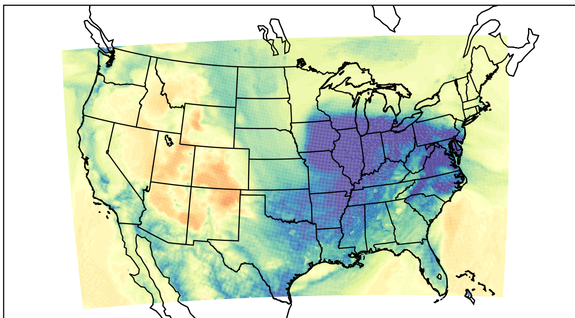
WRF (2019-12-01_11:00:00)
