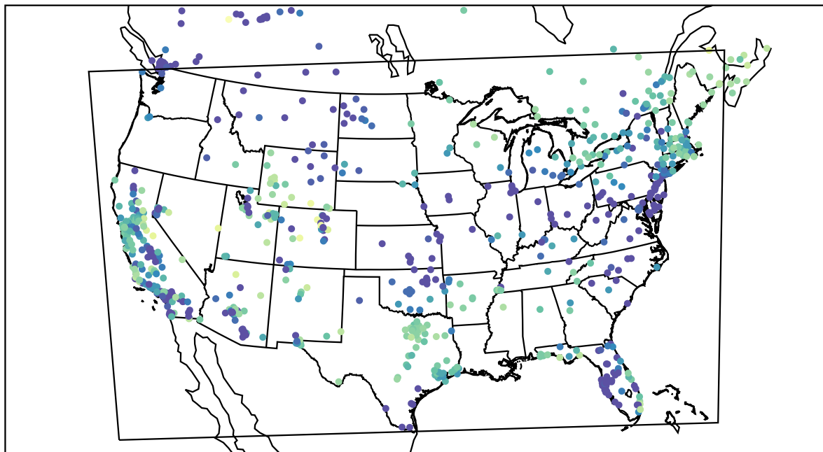
AirNOW (2019-12-01_06:00:00)
