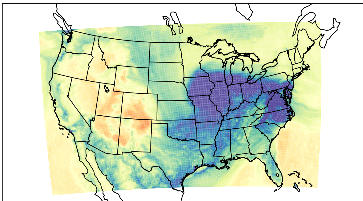
WRF (2019-12-01_09:00:00)
