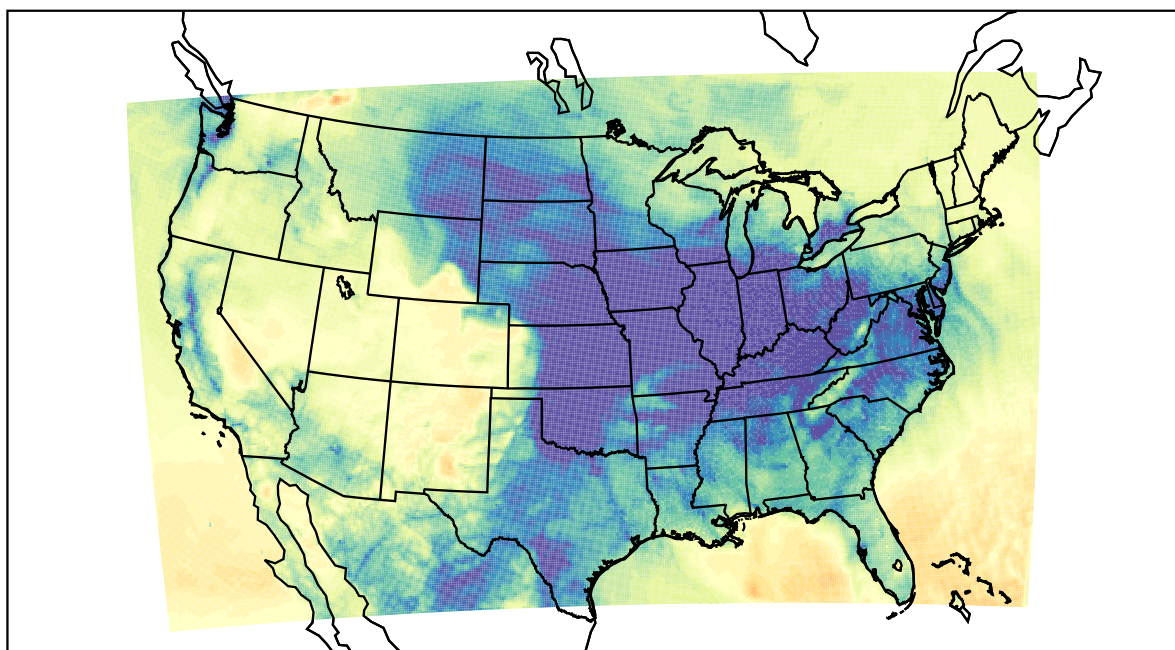
WRF (2019-11-30_06:00:00)
