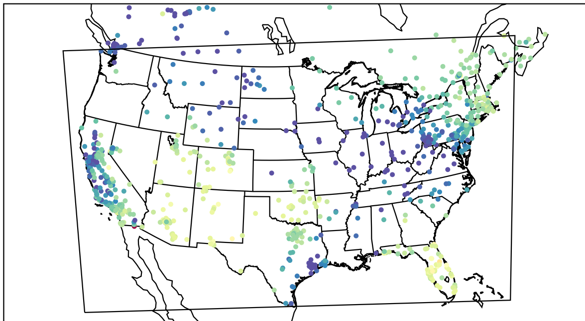
AirNOW (2019-11-30_20:00:00)
