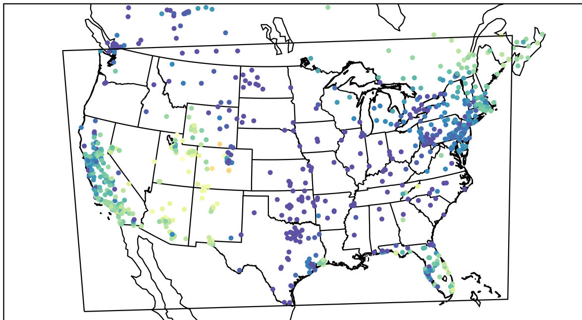
AirNOW (2019-11-30_00:00:00)
