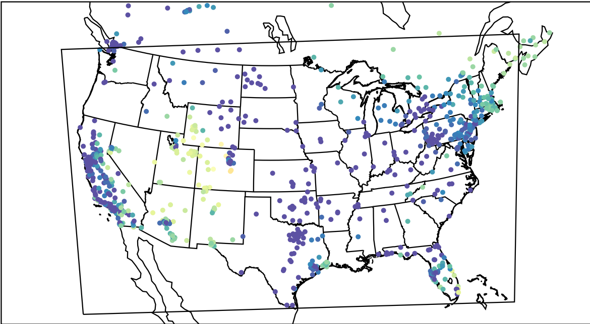
AirNOW (2019-11-30_03:00:00)
