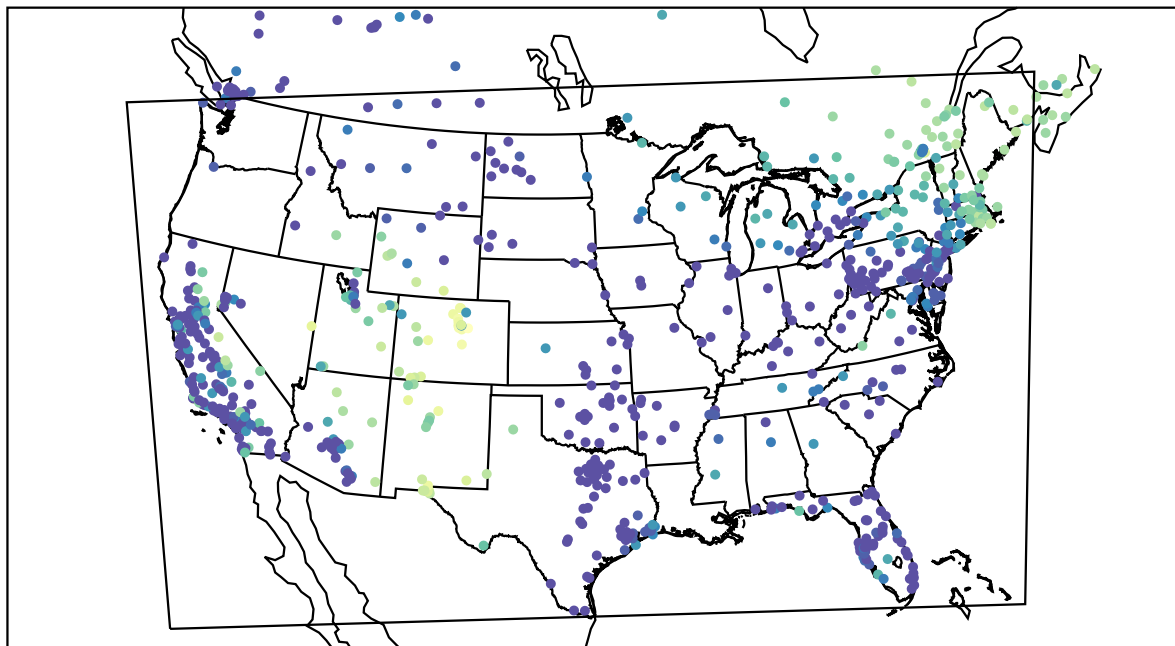
AirNOW (2019-11-30_13:00:00)
