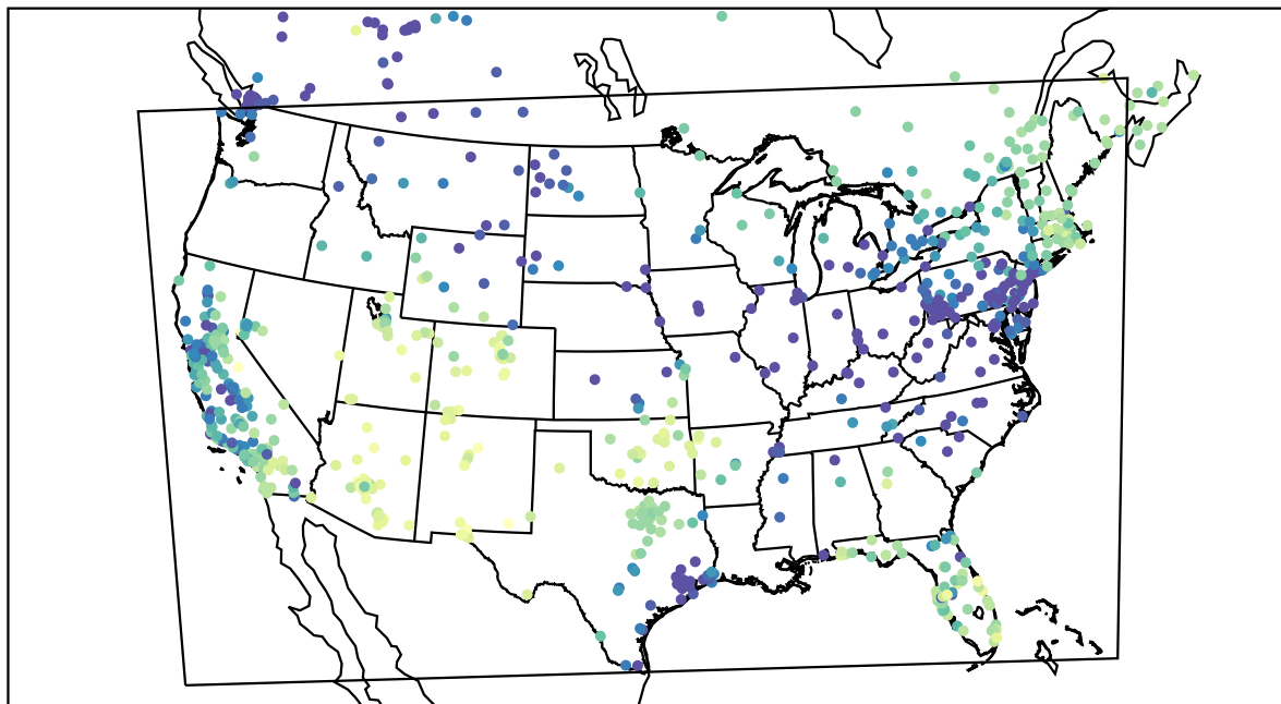
AirNOW (2019-11-30_22:00:00)
