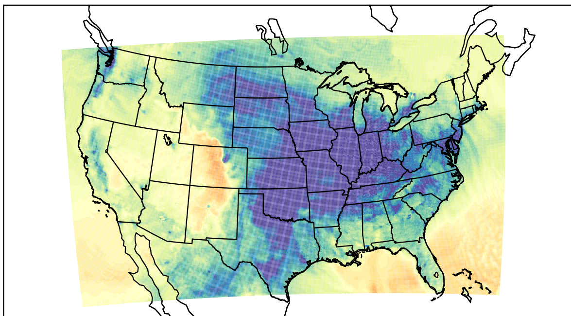
WRF (2019-11-30_01:00:00)
