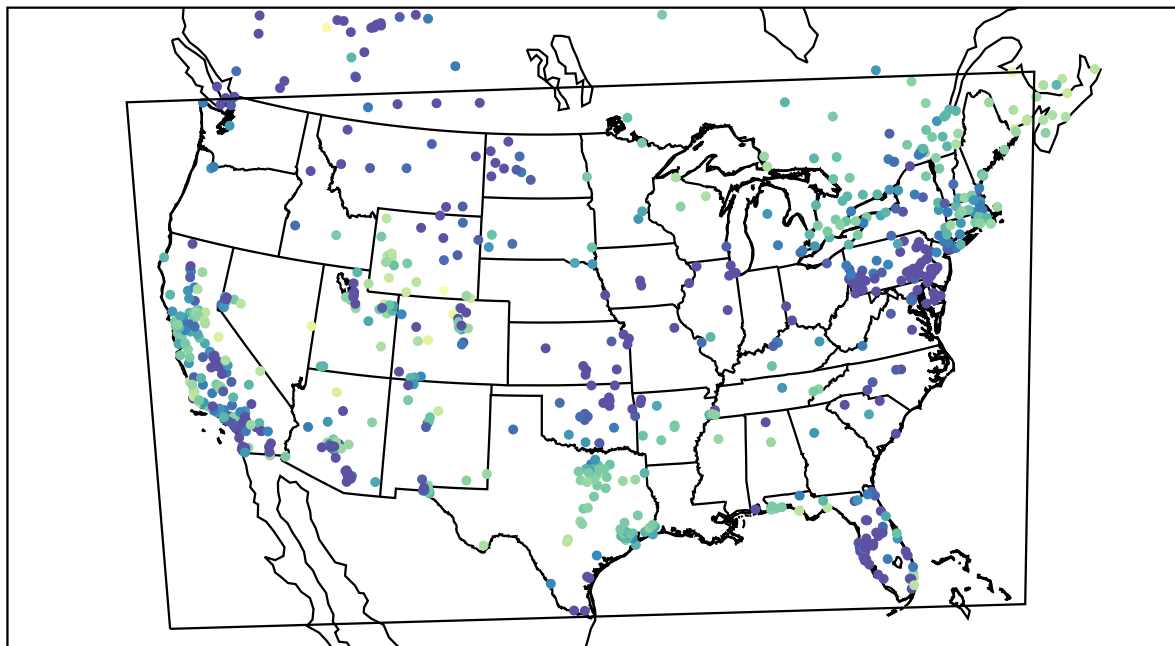
AirNOW (2019-12-01_07:00:00)
