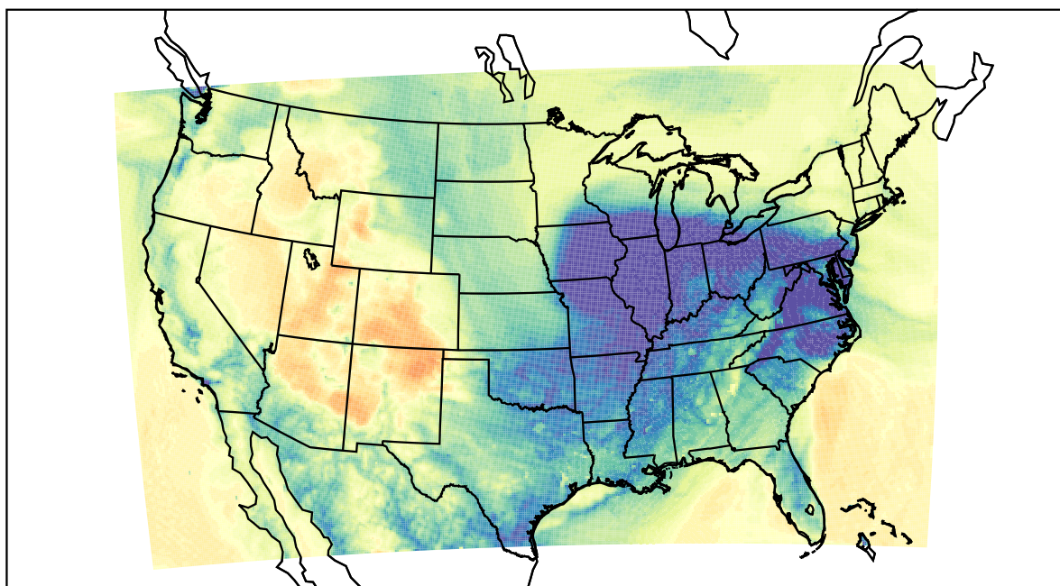
WRF (2019-12-01_10:00:00)
