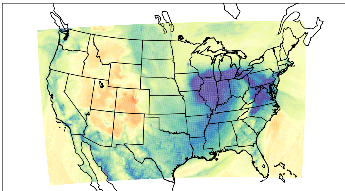
WRF (2019-12-01_15:00:00)
