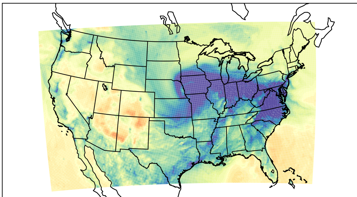
WRF (2019-12-01_04:00:00)
