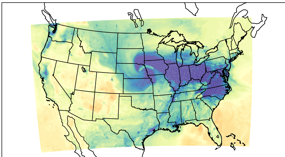
WRF (2019-12-01_00:00:00)
