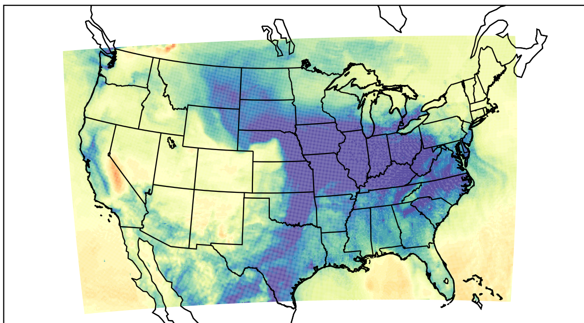
WRF (2019-11-30_12:00:00)
