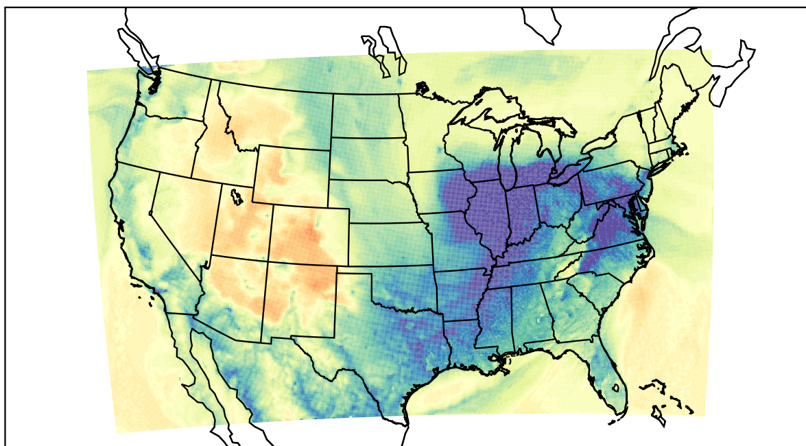
WRF (2019-12-01_14:00:00)
