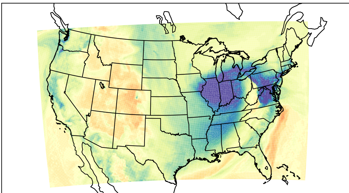
WRF (2019-12-01_19:00:00)
