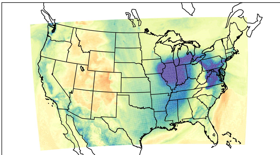
WRF (2019-12-01_17:00:00)
