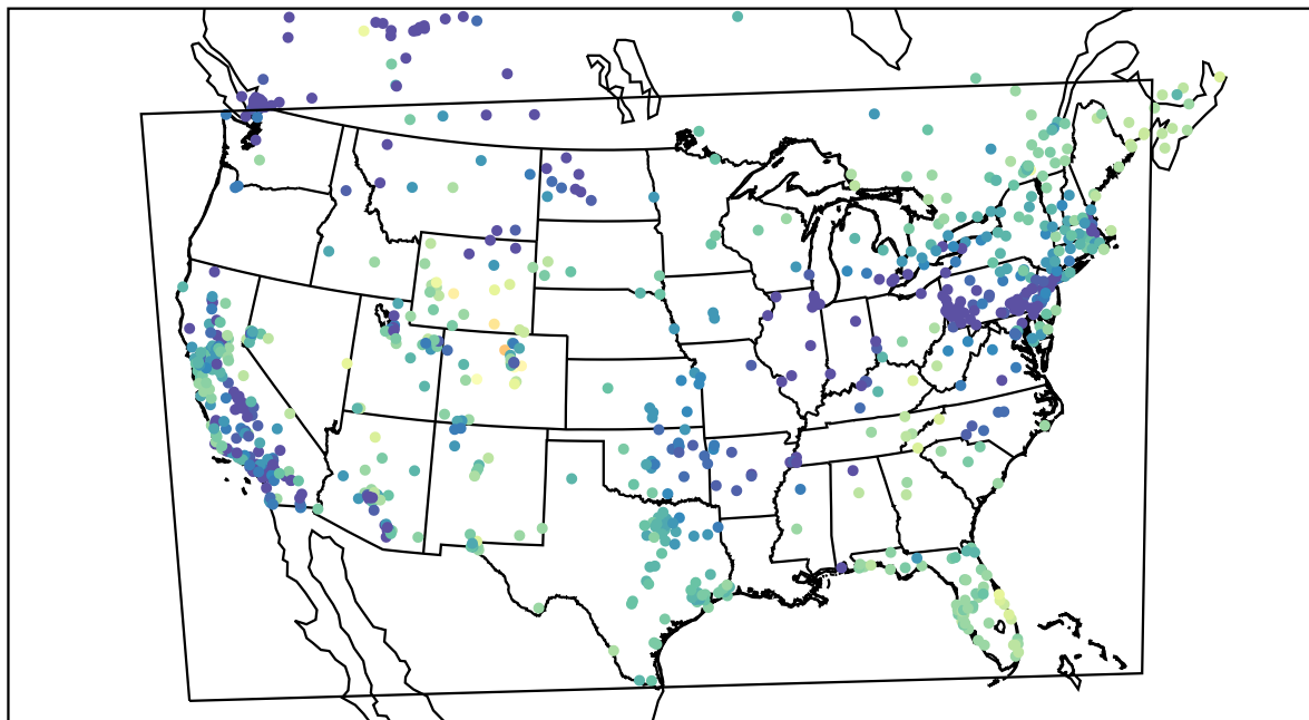
AirNOW (2019-12-01_16:00:00)
