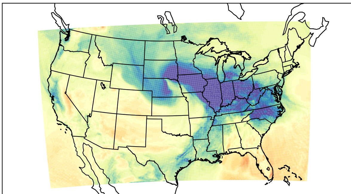
WRF (2019-11-30_19:00:00)
