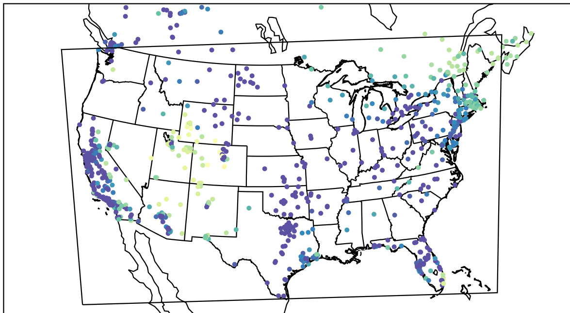
AirNOW (2019-11-30_06:00:00)
