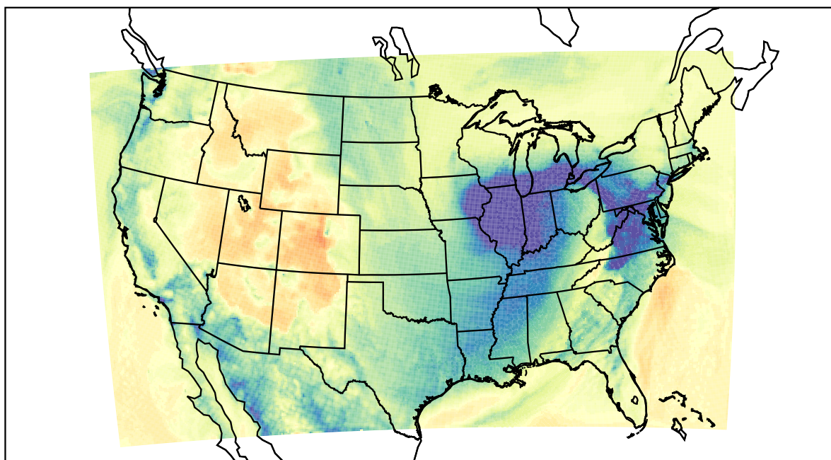
WRF (2019-12-01_16:00:00)
