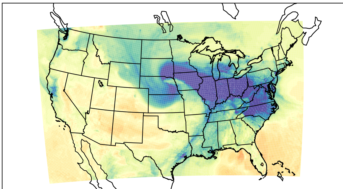
WRF (2019-11-30_22:00:00)
