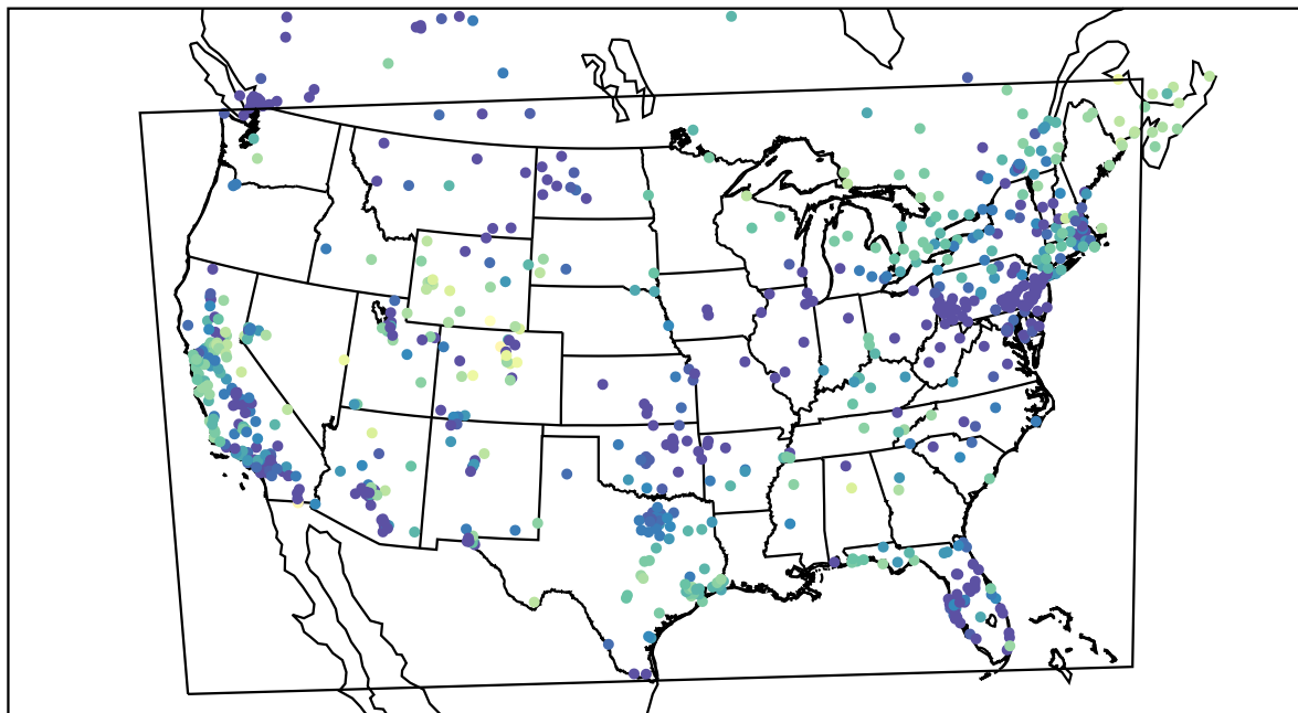
AirNOW (2019-12-01_10:00:00)
