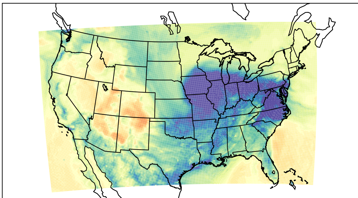
WRF (2019-12-01_08:00:00)
