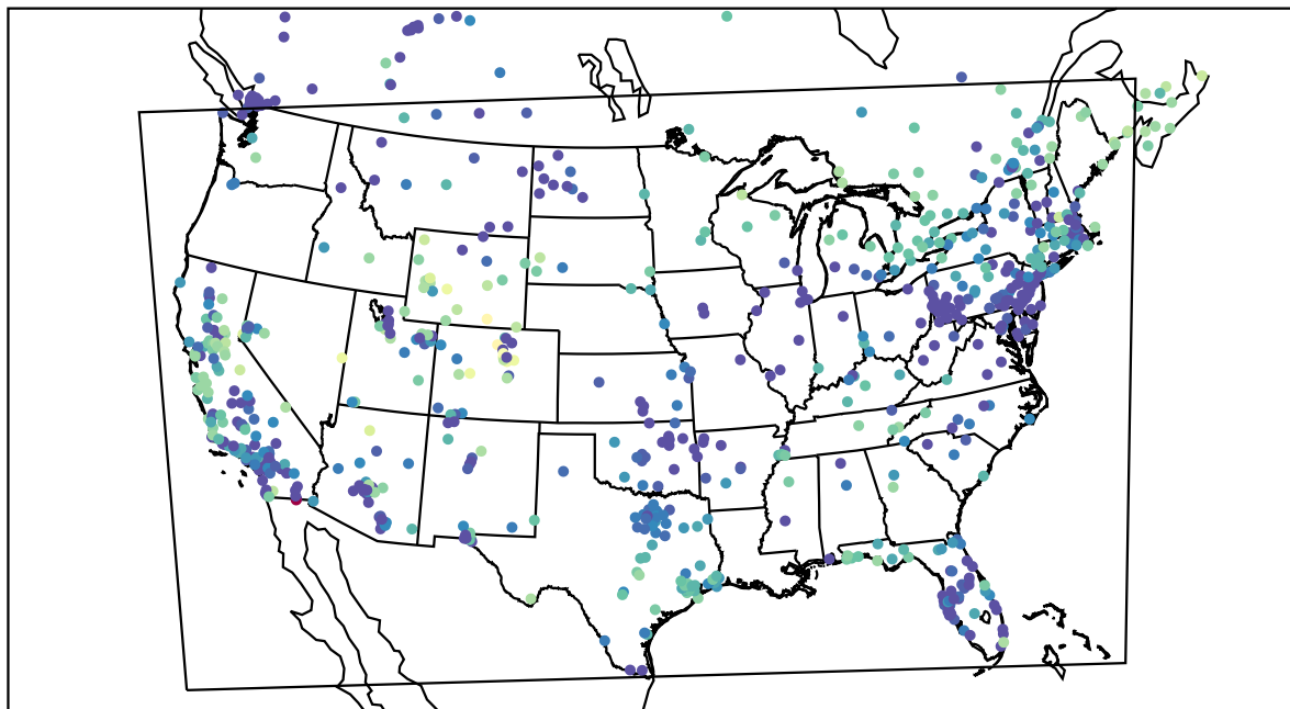
AirNOW (2019-12-01_11:00:00)
