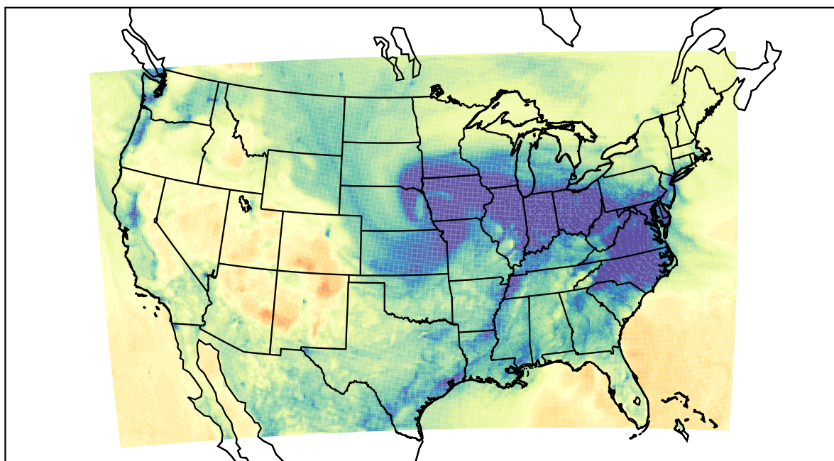
WRF (2019-12-01_02:00:00)
