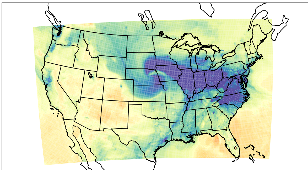
WRF (2019-11-30_23:00:00)
