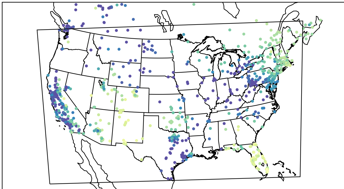
AirNOW (2019-11-30_17:00:00)
