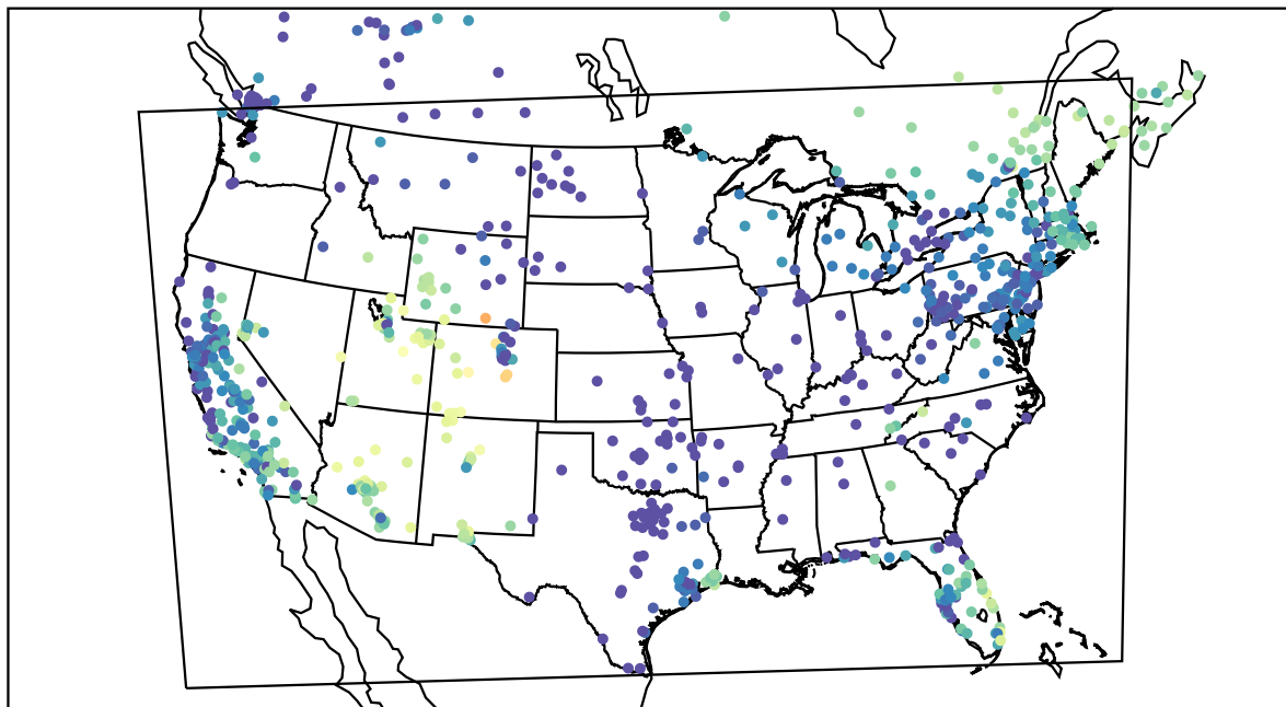
AirNOW (2019-11-30_01:00:00)
