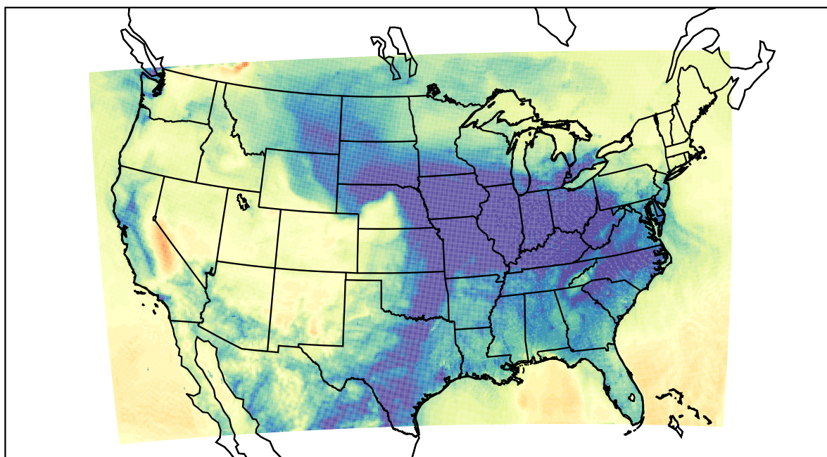
WRF (2019-11-30_13:00:00)
