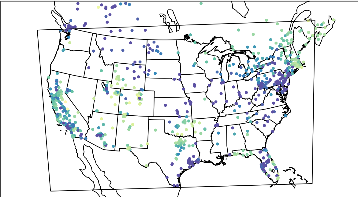
AirNOW (2019-12-01_01:00:00)
