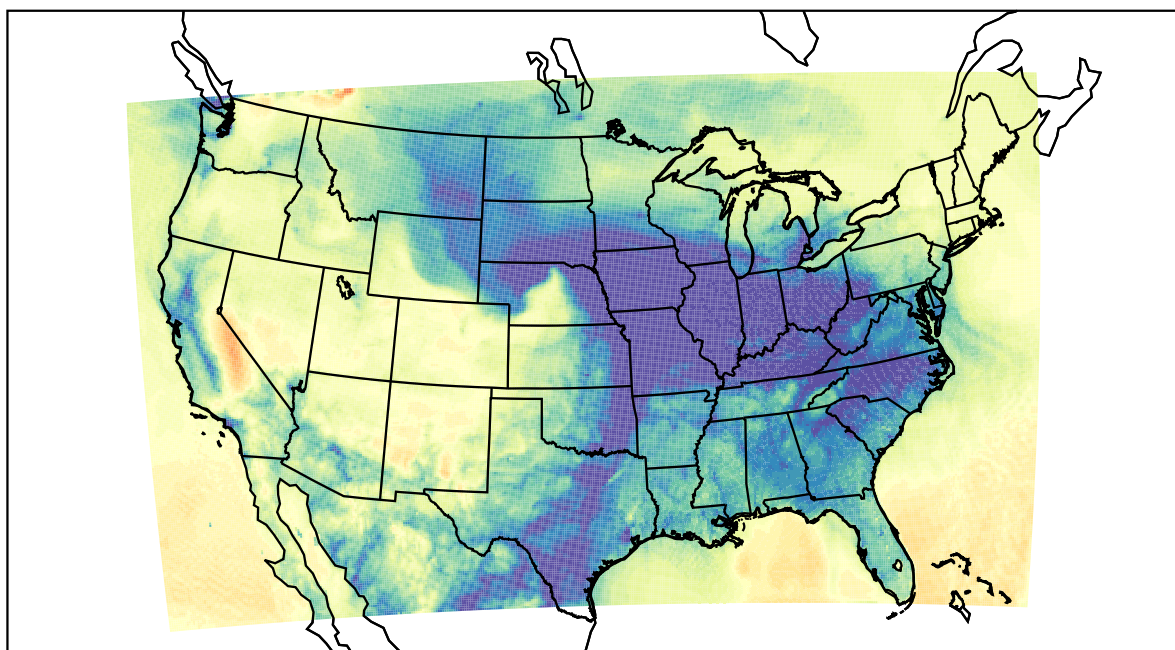
WRF (2019-11-30_14:00:00)
