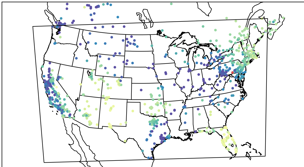
AirNOW (2019-11-30_18:00:00)
