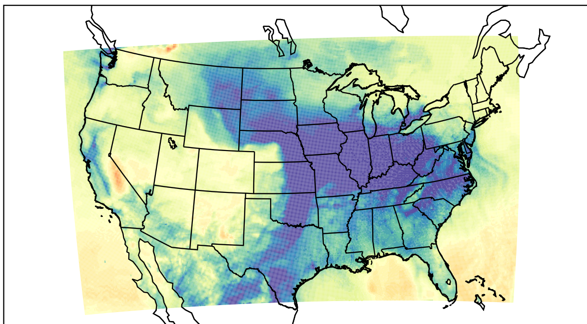
WRF (2019-11-30_11:00:00)
