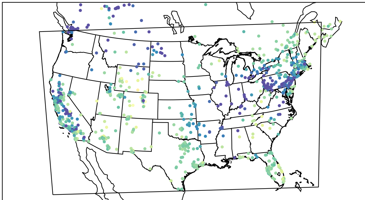
AirNOW (2019-12-01_18:00:00)
