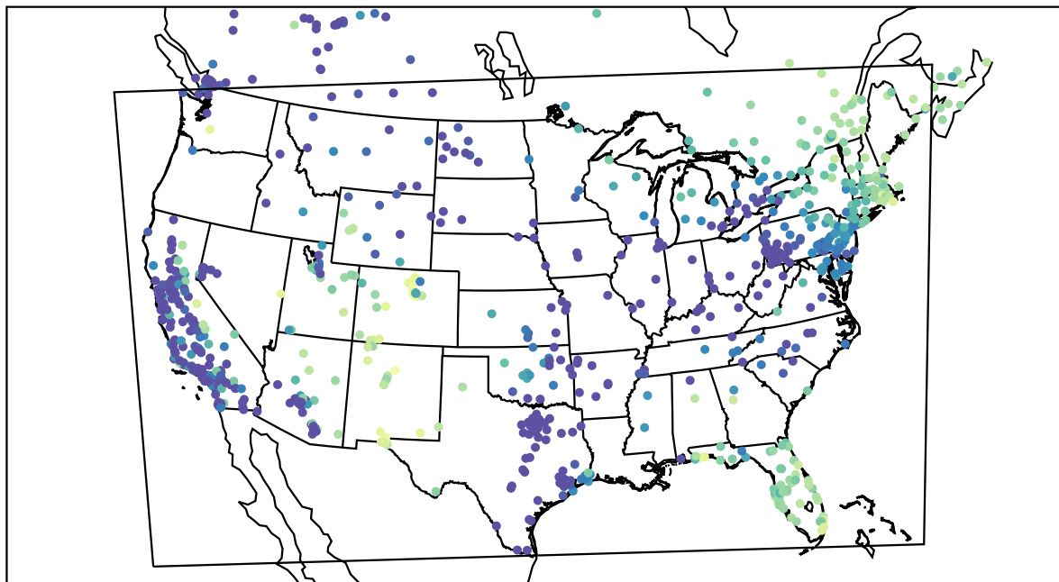
AirNOW (2019-11-30_15:00:00)
