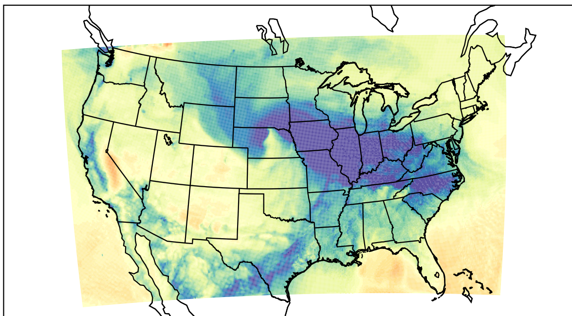
WRF (2019-11-30_16:00:00)
