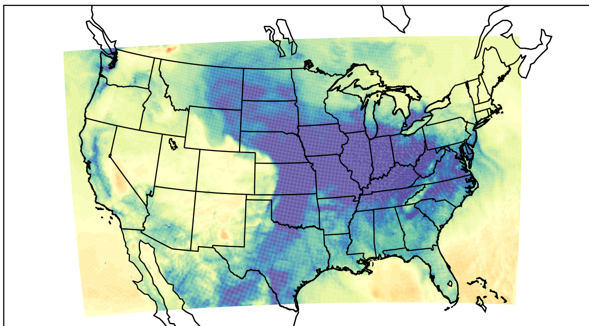
WRF (2019-11-30_08:00:00)
