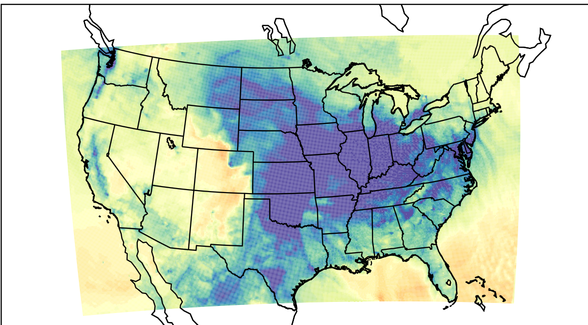
WRF (2019-11-30_03:00:00)
