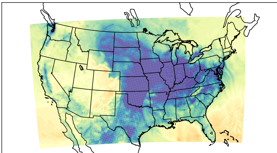
WRF (2019-11-30_04:00:00)
