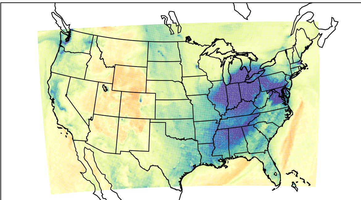
WRF (2019-12-01_23:00:00)
