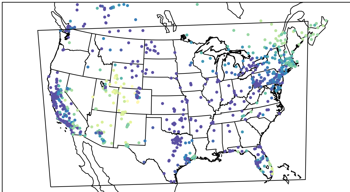
AirNOW (2019-11-30_04:00:00)
