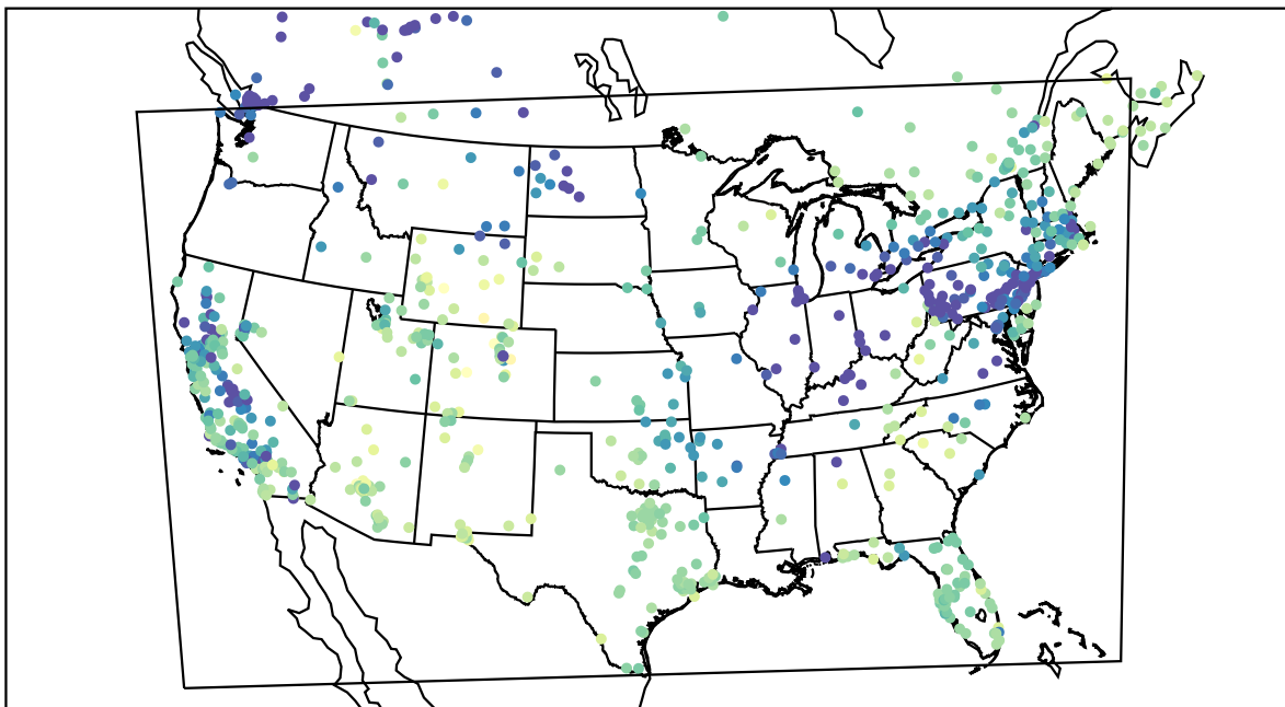
AirNOW (2019-12-01_19:00:00)
