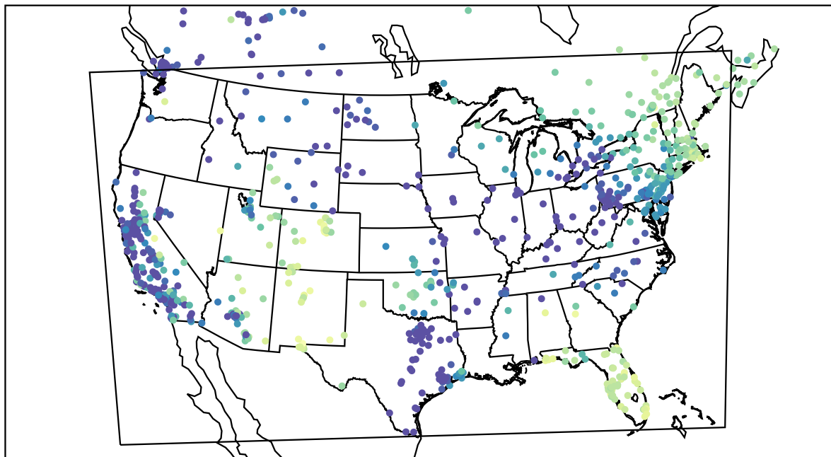
AirNOW (2019-11-30_16:00:00)
