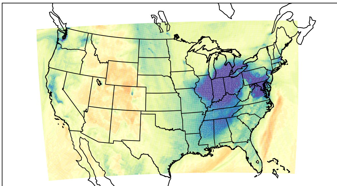
WRF (2019-12-01_22:00:00)
