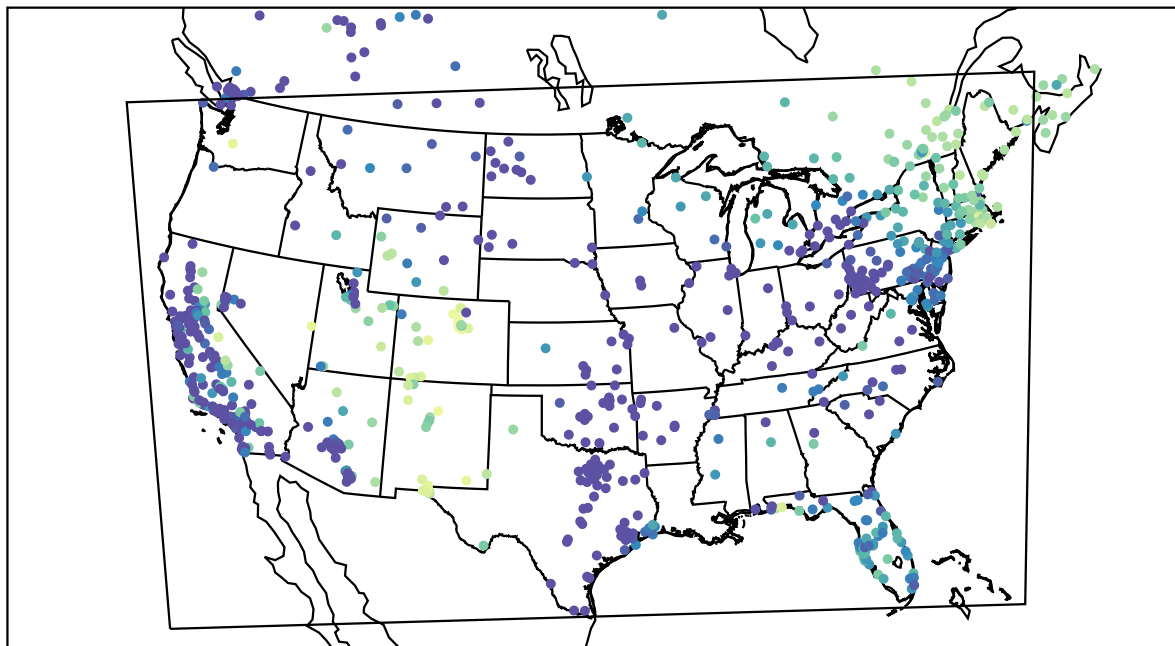
AirNOW (2019-11-30_14:00:00)
