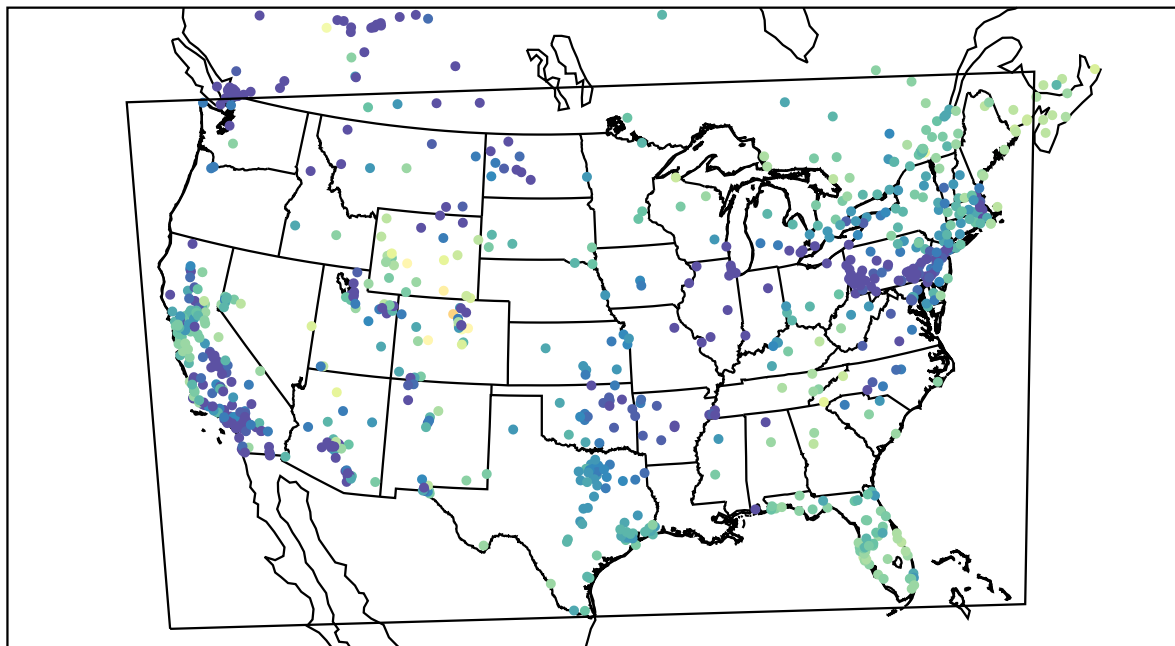
AirNOW (2019-12-01_15:00:00)
