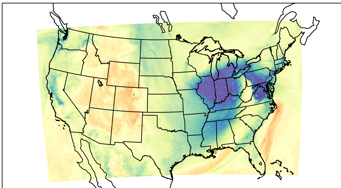
WRF (2019-12-01_20:00:00)
