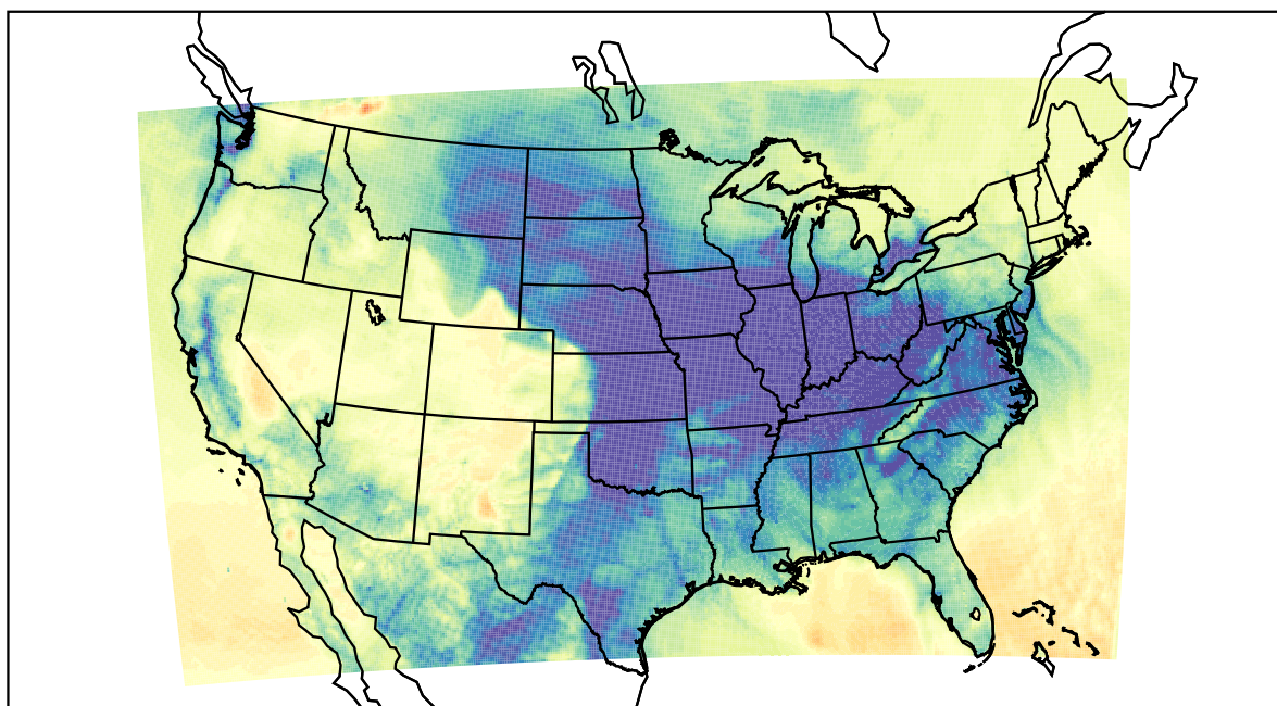
WRF (2019-11-30_07:00:00)
