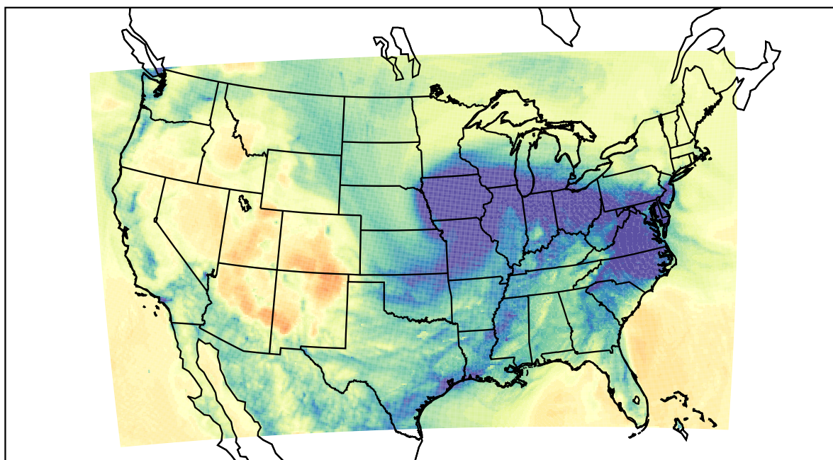
WRF (2019-12-01_06:00:00)
