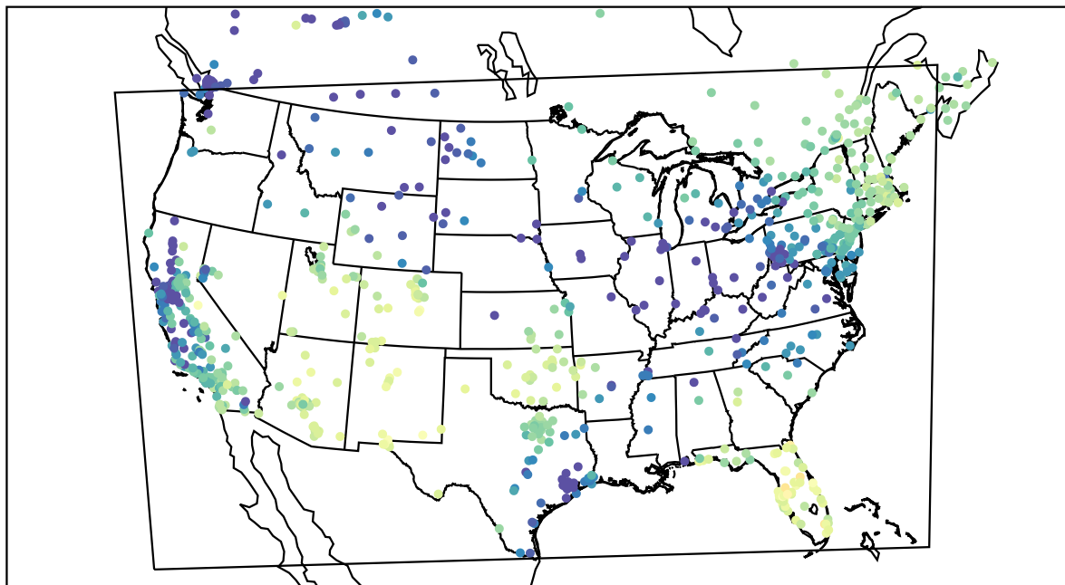
AirNOW (2019-11-30_19:00:00)
