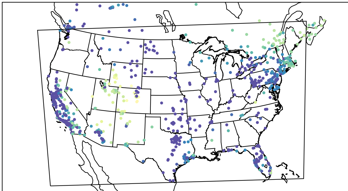
AirNOW (2019-11-30_07:00:00)
