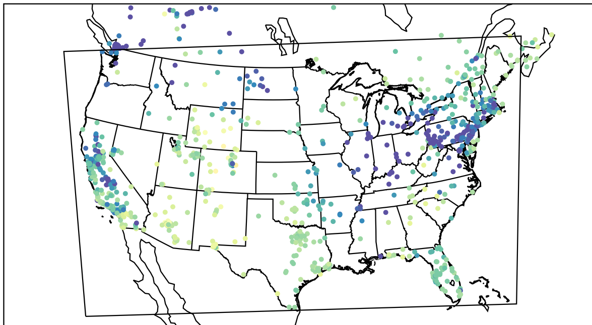
AirNOW (2019-12-01_20:00:00)
