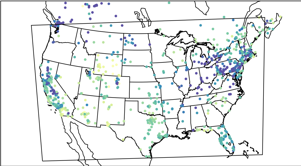
AirNOW (2019-12-01_23:00:00)
