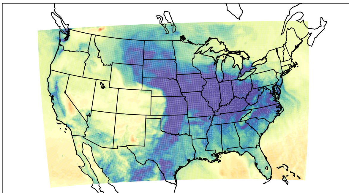
WRF (2019-11-30_09:00:00)
