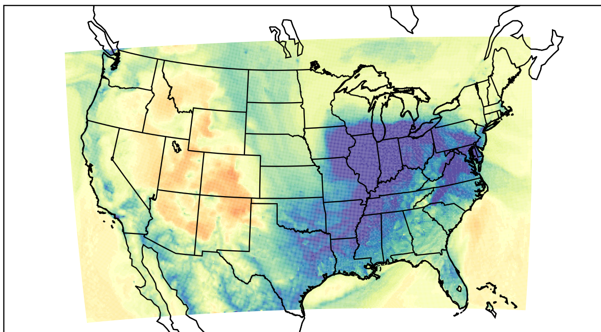
WRF (2019-12-01_13:00:00)
