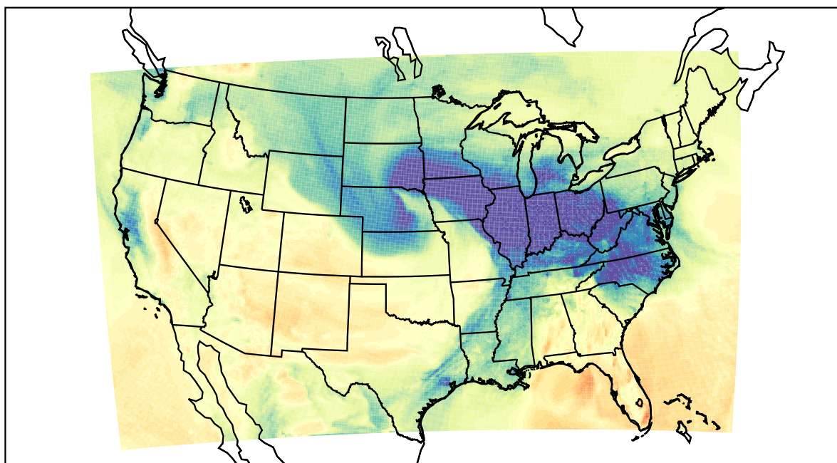
WRF (2019-11-30_20:00:00)
