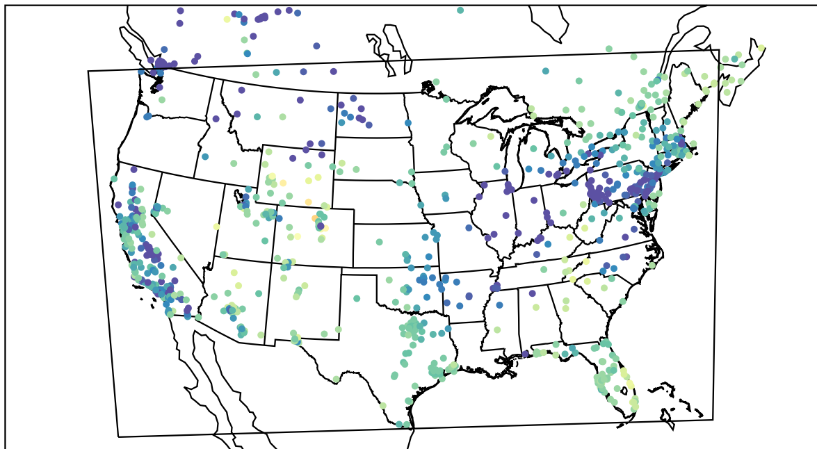
AirNOW (2019-12-01_17:00:00)
