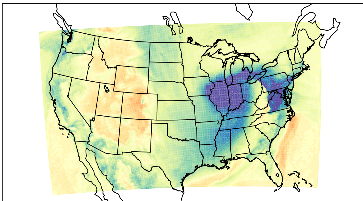
WRF (2019-12-01_18:00:00)
