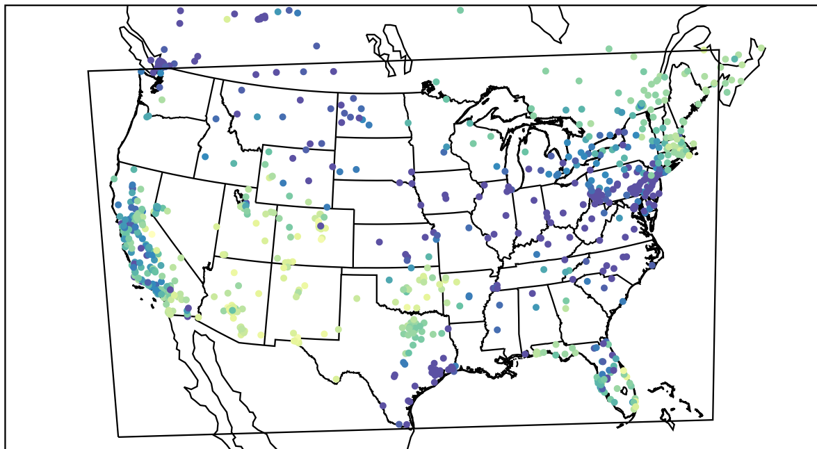
AirNOW (2019-11-30_23:00:00)
