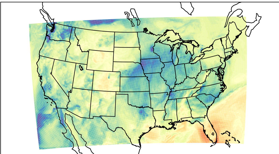
WRF (2019-12-07_20:00:00)
