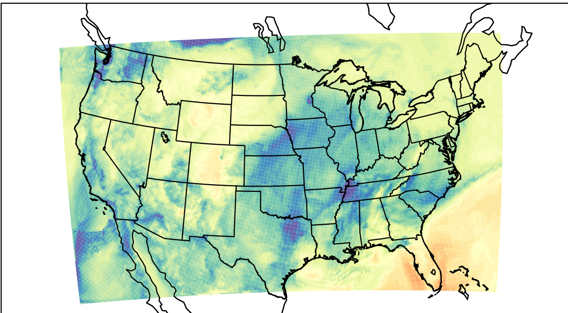
WRF (2019-12-07_18:00:00)
