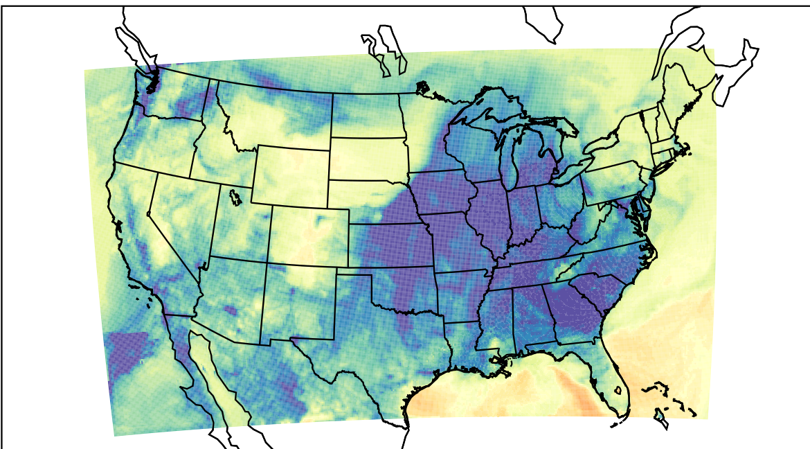
WRF (2019-12-08_06:00:00)
