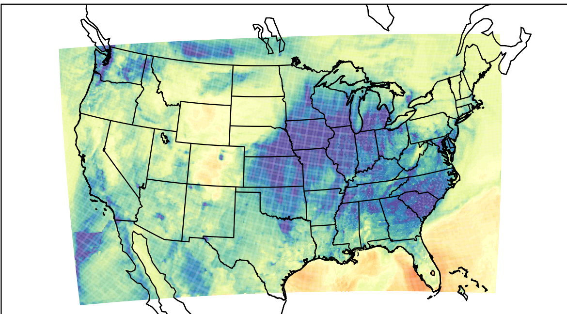
WRF (2019-12-08_00:00:00)
