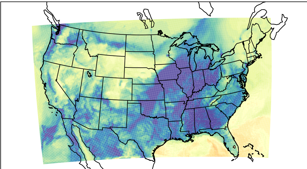
WRF (2019-12-08_14:00:00)
