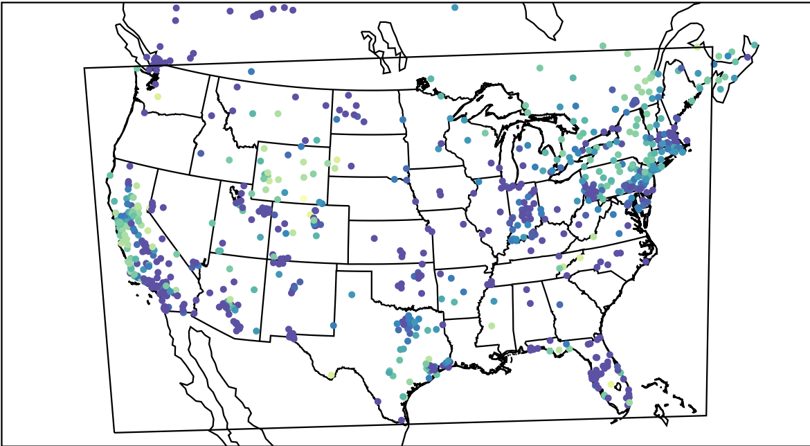
AirNOW (2019-12-07_04:00:00)
