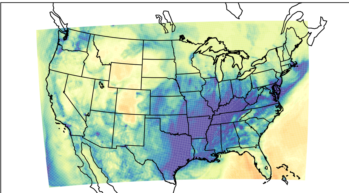
WRF (2019-12-07_06:00:00)
