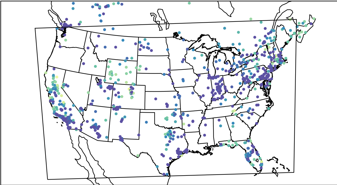
AirNOW (2019-12-08_11:00:00)
