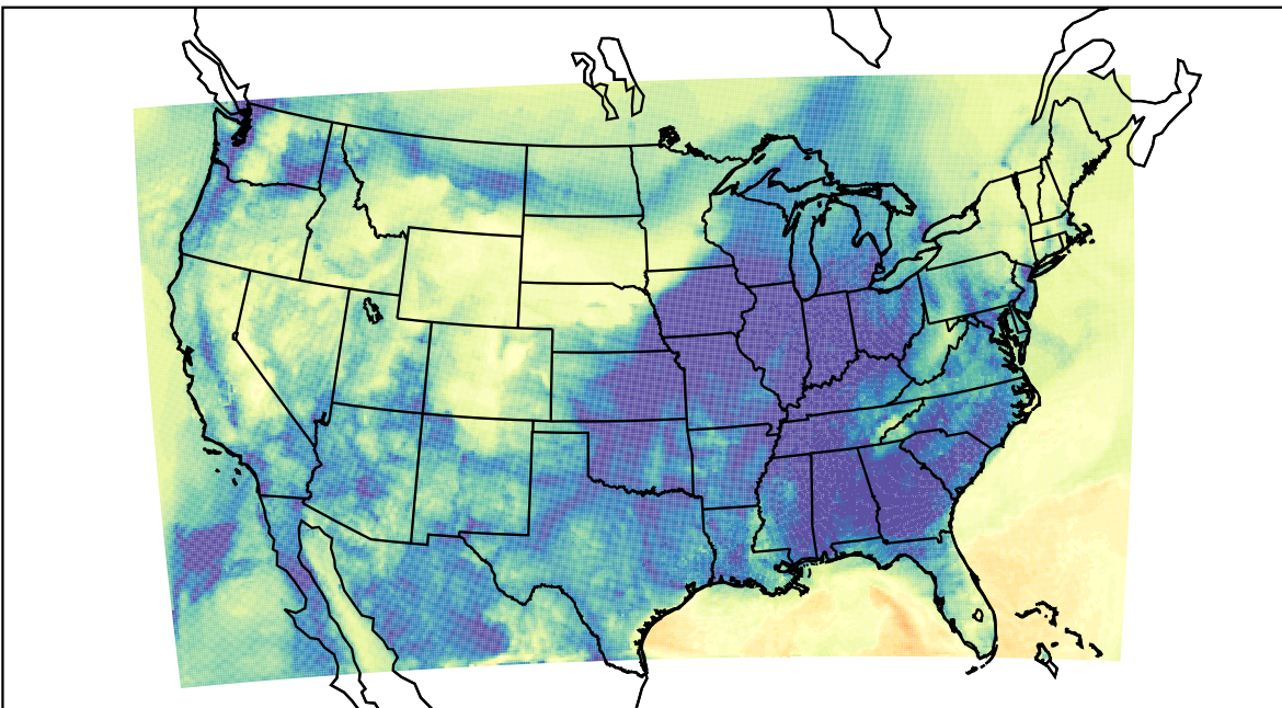
WRF (2019-12-08_12:00:00)
