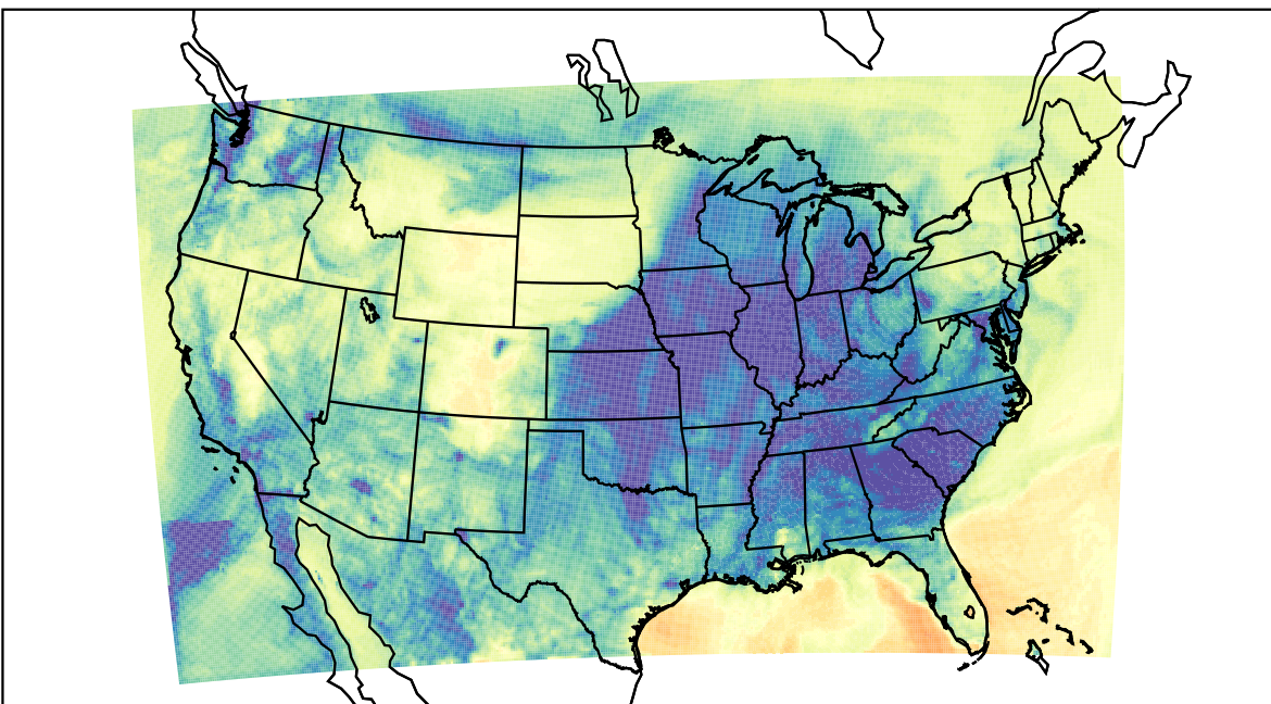
WRF (2019-12-08_04:00:00)
