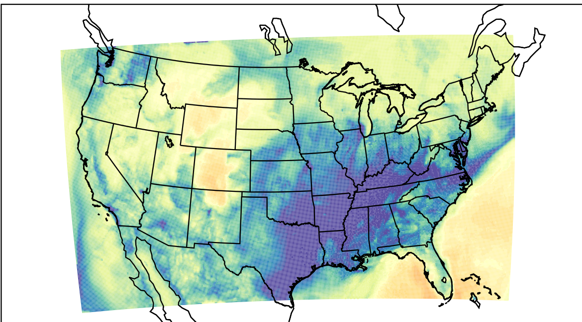
WRF (2019-12-07_09:00:00)
