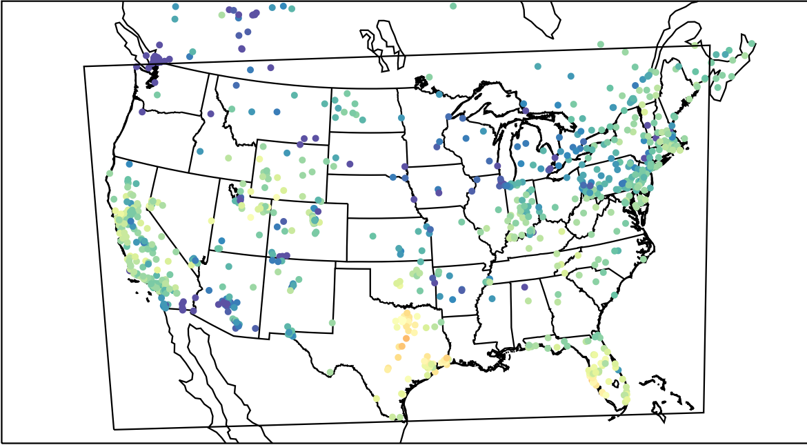
AirNOW (2019-12-08_20:00:00)
