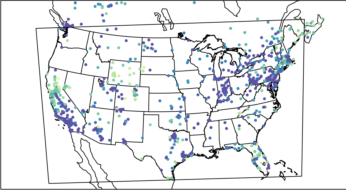
AirNOW (2019-12-08_03:00:00)
