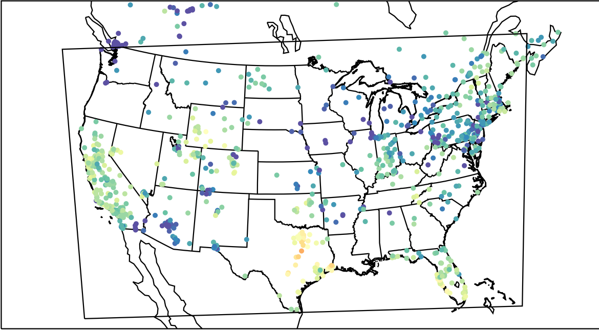
AirNOW (2019-12-08_22:00:00)
