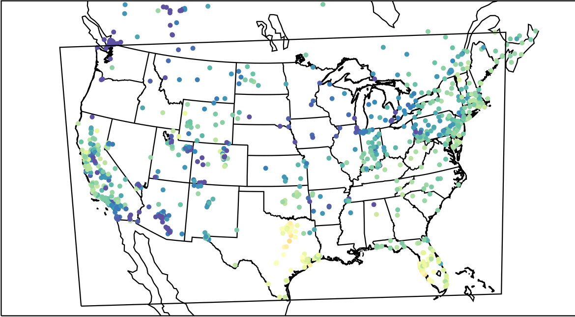
AirNOW (2019-12-08_18:00:00)
