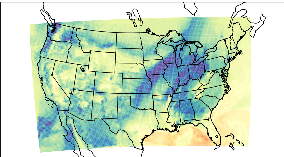
WRF (2019-12-08_18:00:00)
