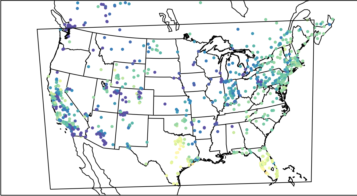
AirNOW (2019-12-08_17:00:00)
