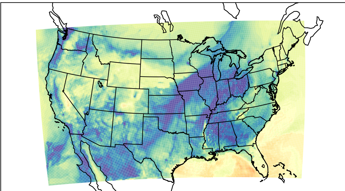
WRF (2019-12-08_16:00:00)
