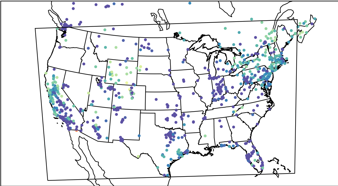
AirNOW (2019-12-07_08:00:00)
