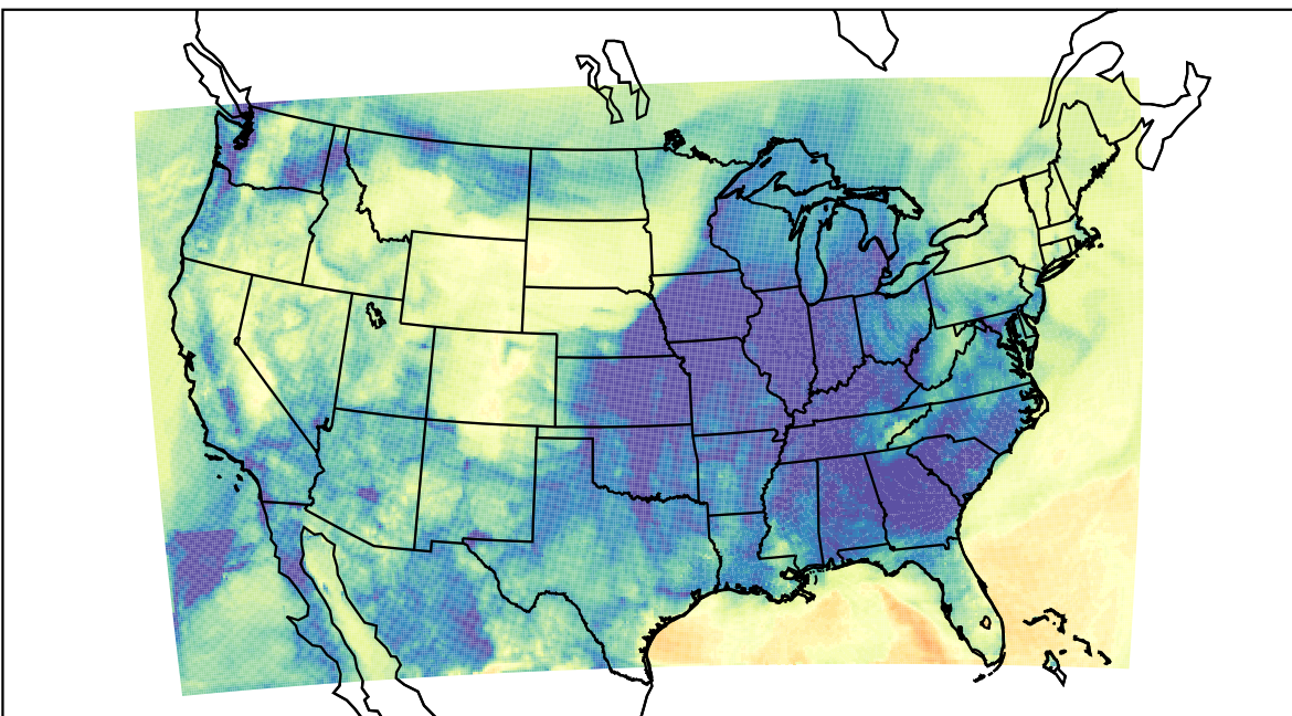
WRF (2019-12-08_08:00:00)
