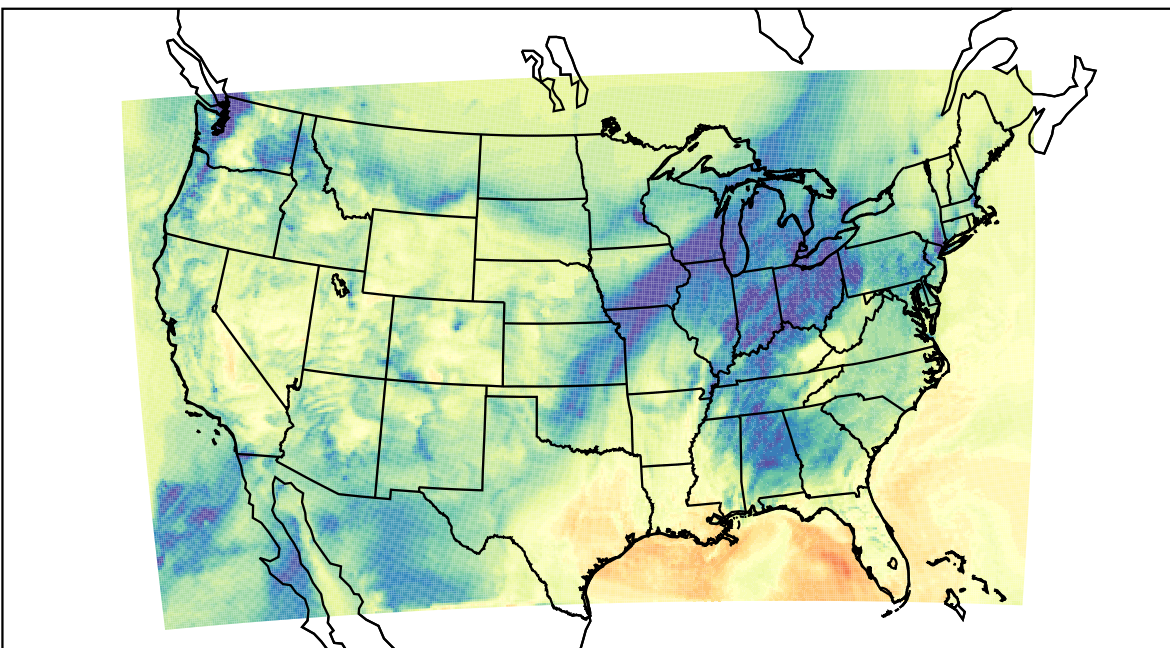
WRF (2019-12-08_20:00:00)
