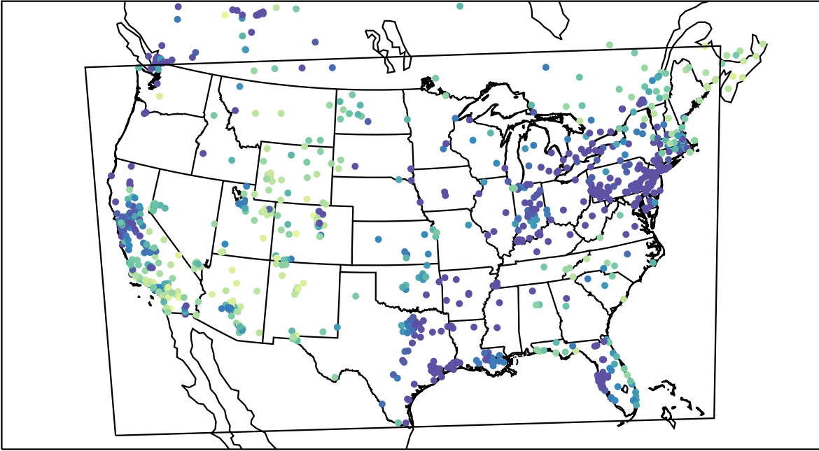
AirNOW (2019-12-17_00:00:00)
