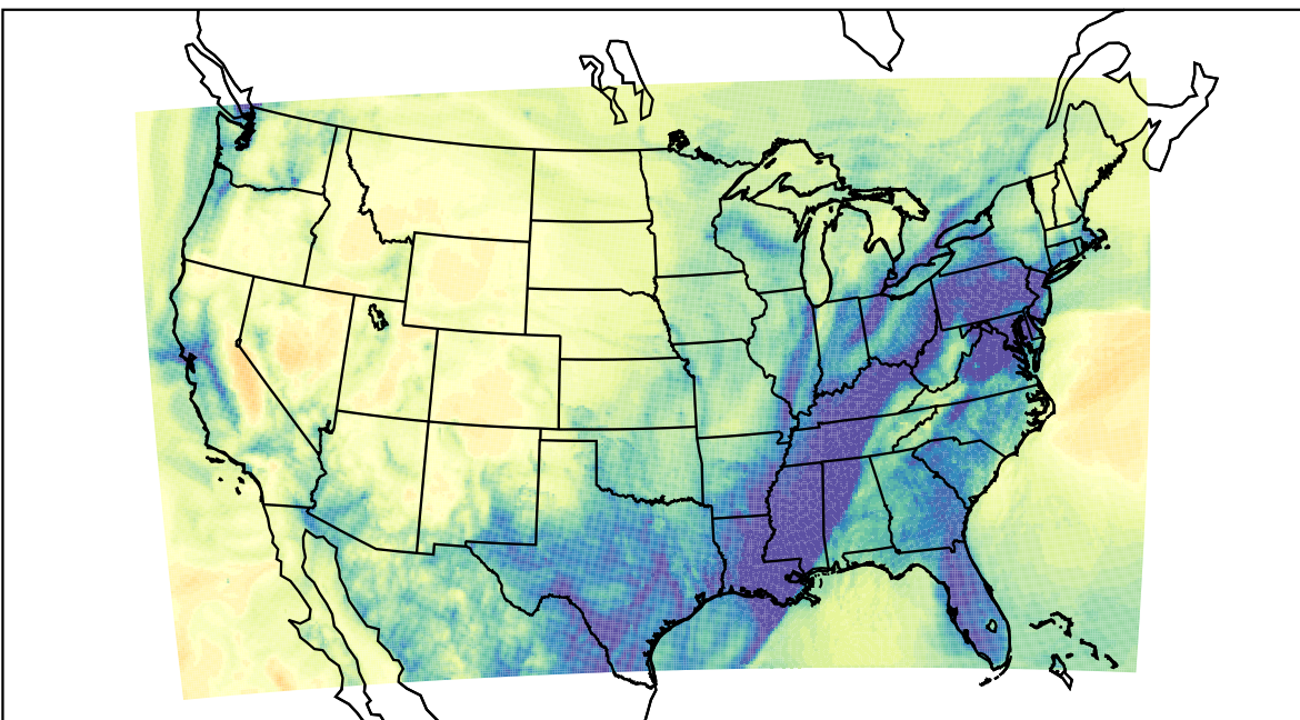
WRF (2019-12-17_08:00:00)
