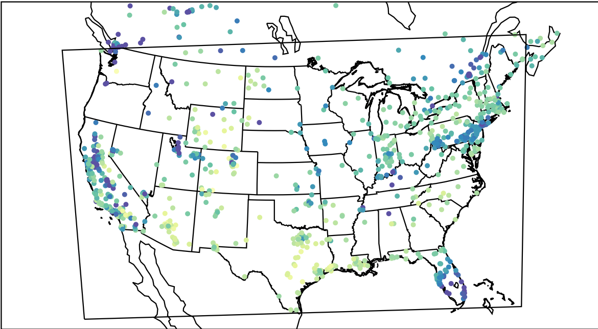
AirNOW (2019-12-18_19:00:00)
