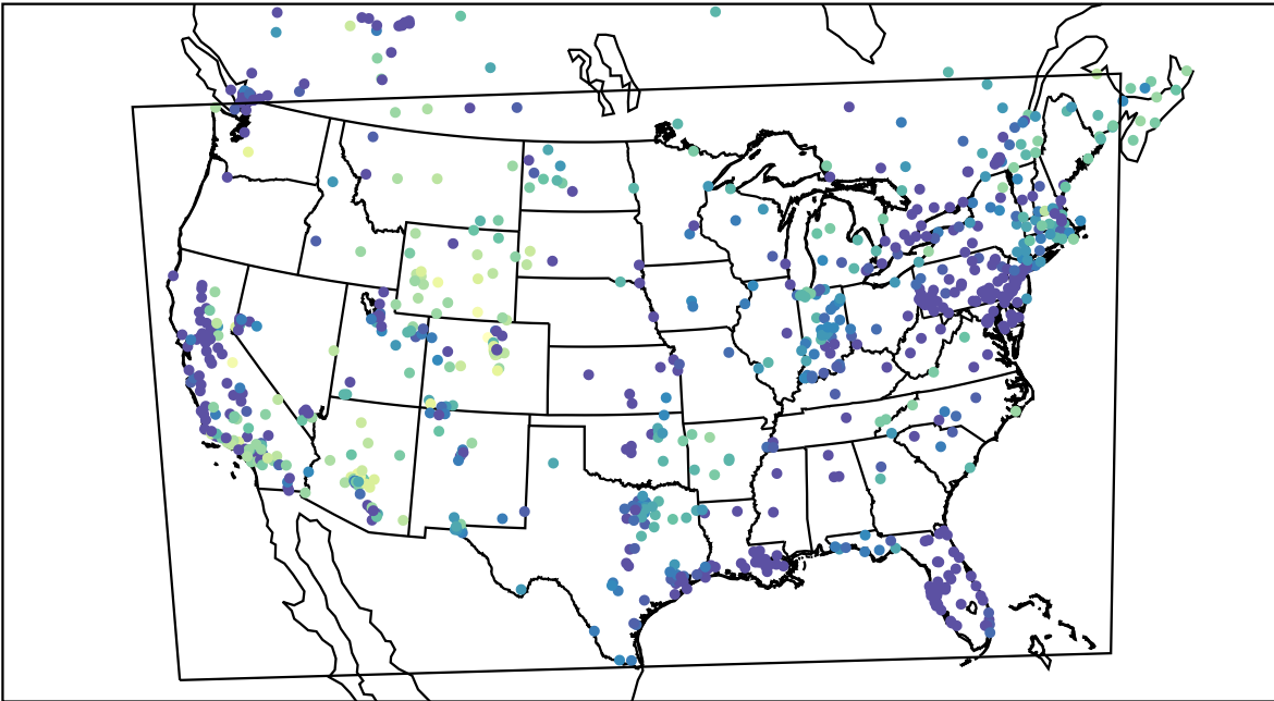
AirNOW (2019-12-17_11:00:00)
