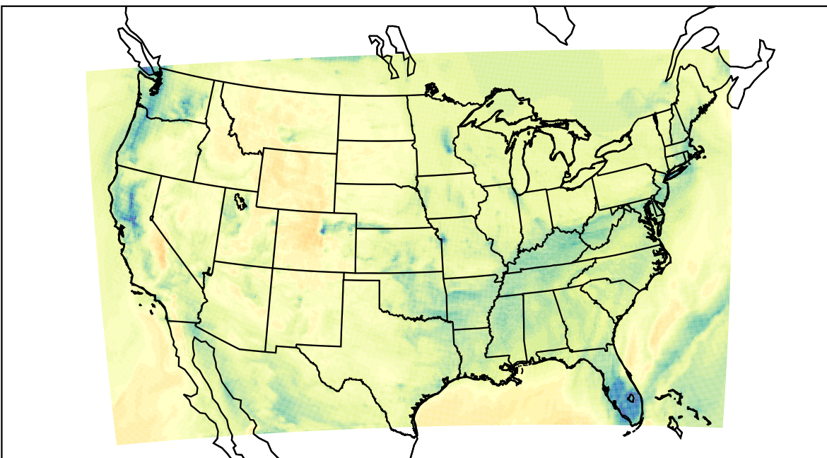
WRF (2019-12-18_20:00:00)
