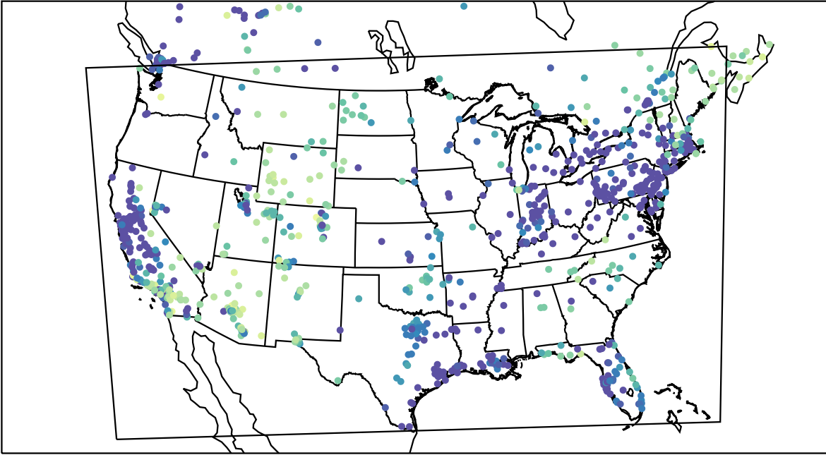
AirNOW (2019-12-17_03:00:00)
