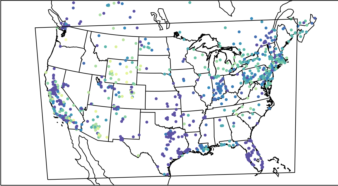
AirNOW (2019-12-18_10:00:00)
