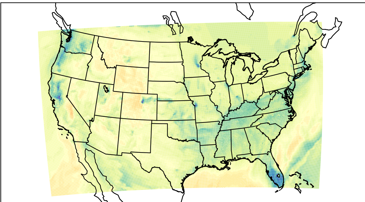
WRF (2019-12-18_21:00:00)
