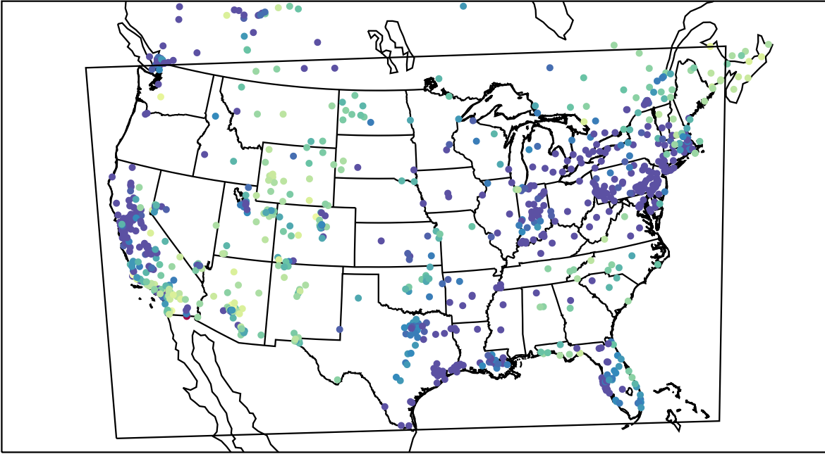
AirNOW (2019-12-17_02:00:00)
