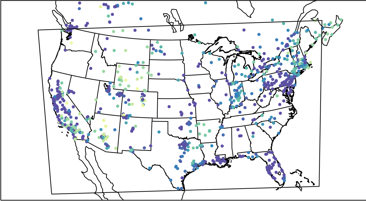
AirNOW (2019-12-17_14:00:00)
