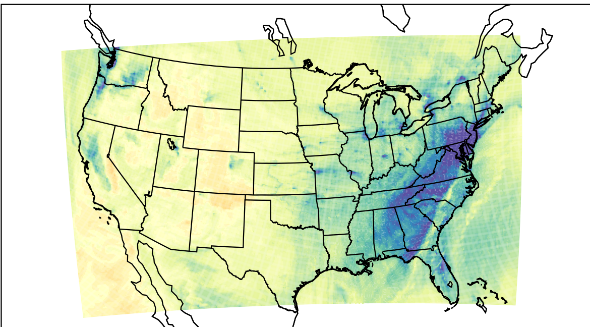
WRF (2019-12-17_22:00:00)
