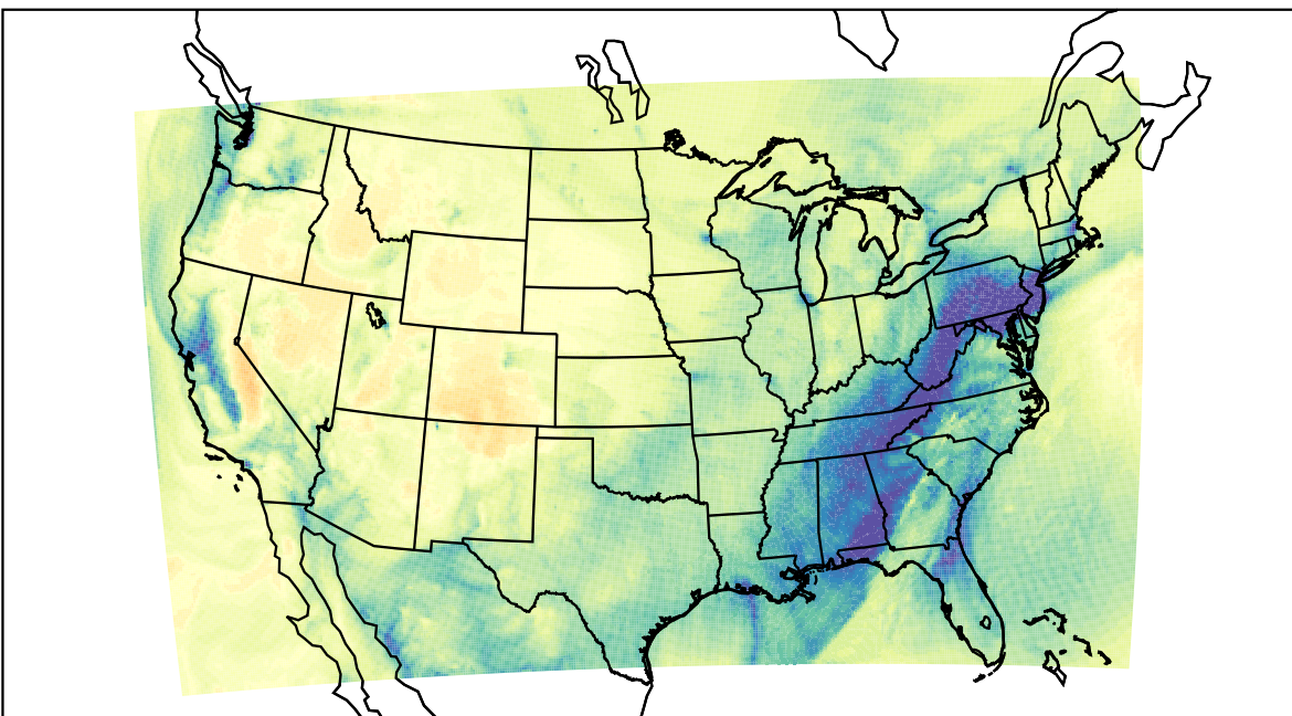
WRF (2019-12-17_17:00:00)
