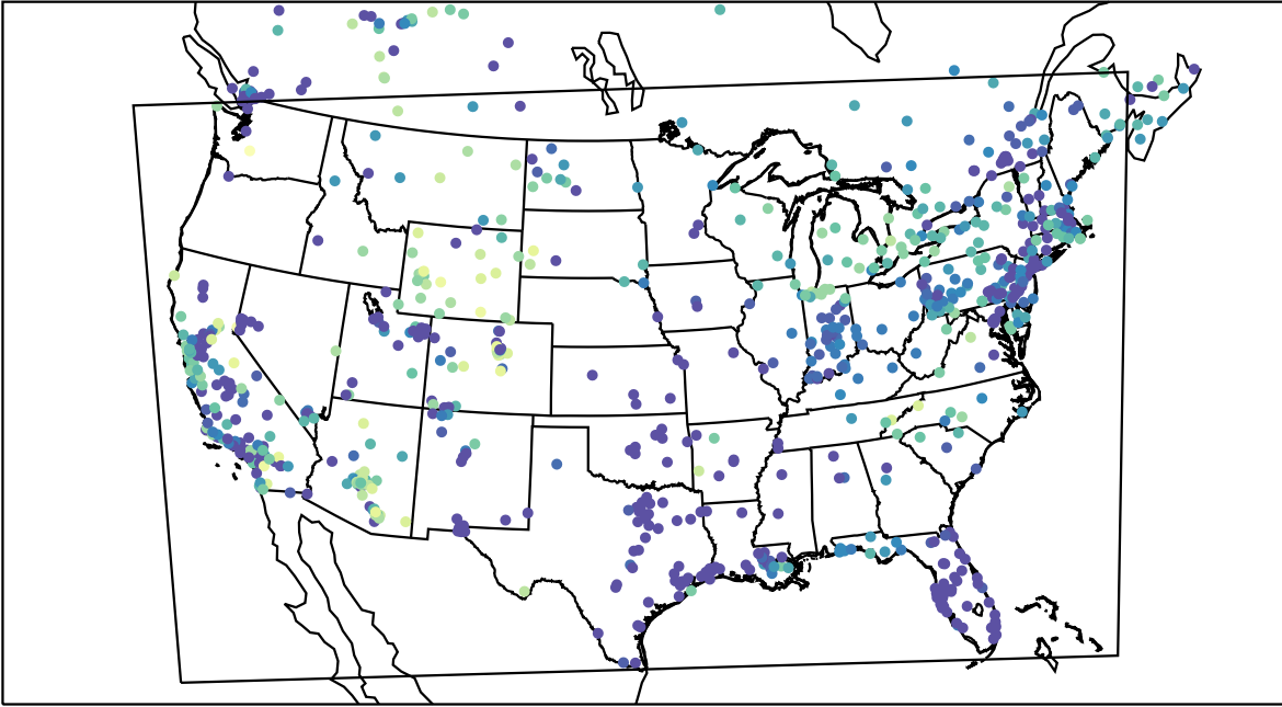
AirNOW (2019-12-18_12:00:00)
