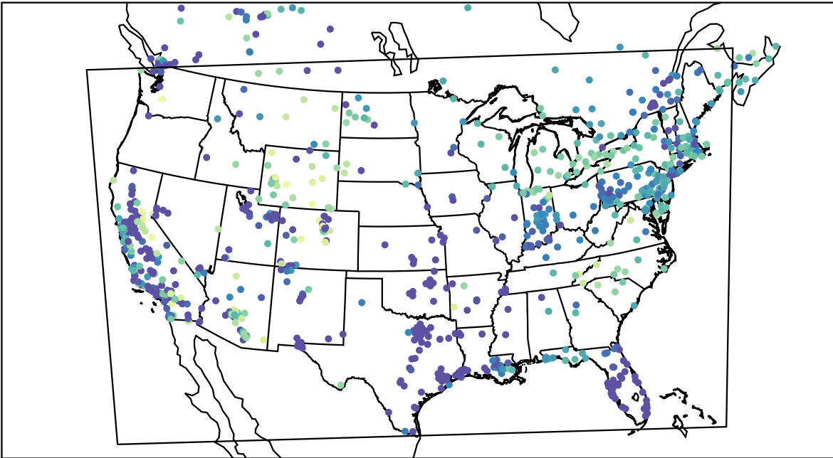
AirNOW (2019-12-18_14:00:00)
