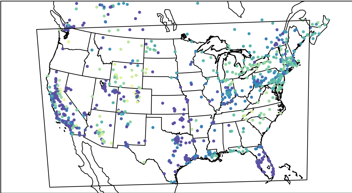
AirNOW (2019-12-18_15:00:00)
