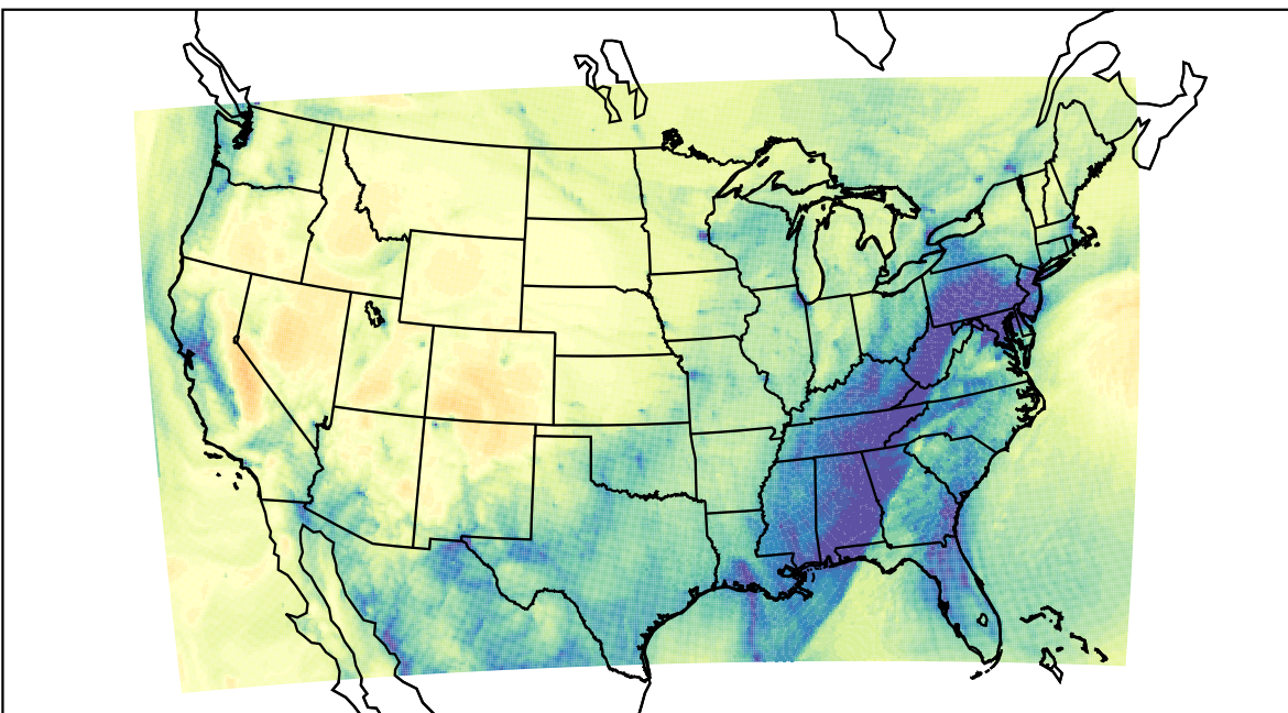
WRF (2019-12-17_15:00:00)
