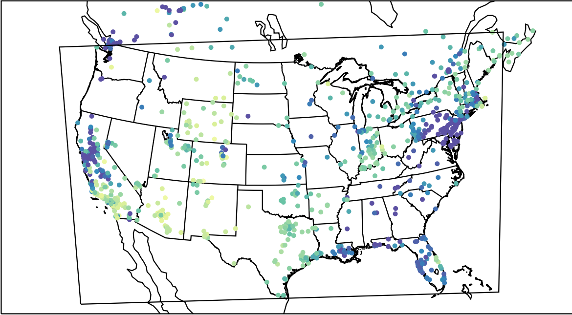
AirNOW (2019-12-17_19:00:00)
