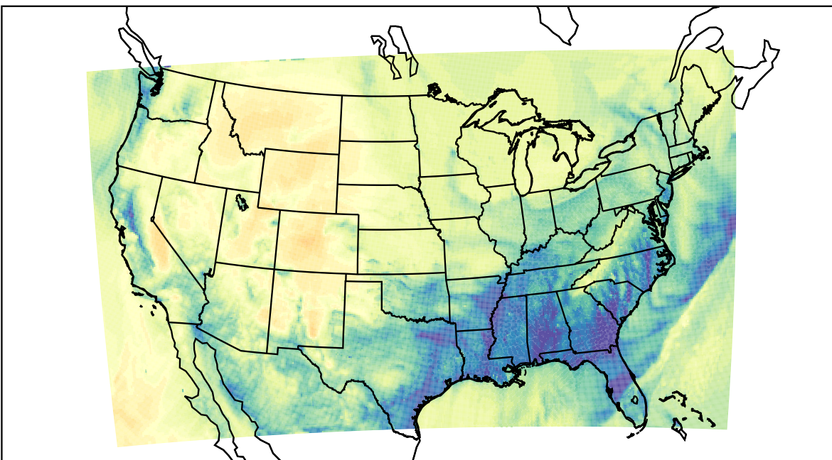
WRF (2019-12-18_10:00:00)
