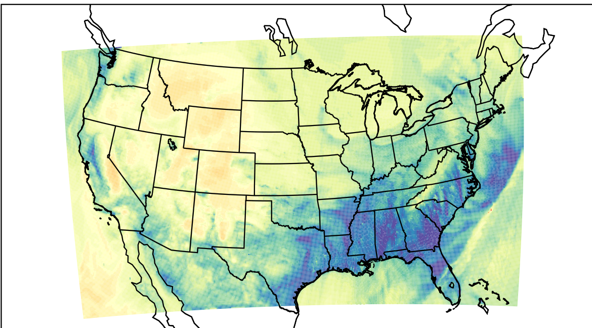
WRF (2019-12-18_08:00:00)
