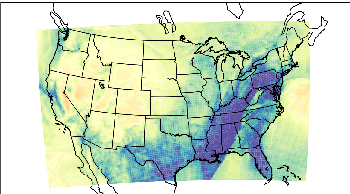
WRF (2019-12-17_12:00:00)
