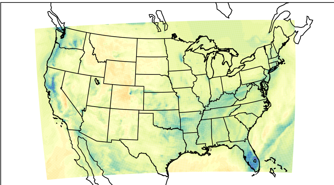
WRF (2019-12-18_19:00:00)
