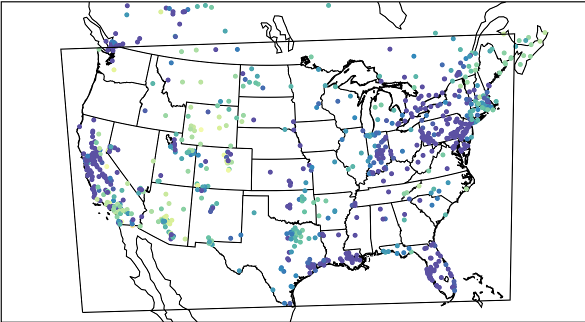
AirNOW (2019-12-17_09:00:00)
