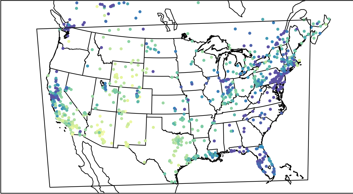
AirNOW (2019-12-17_22:00:00)
