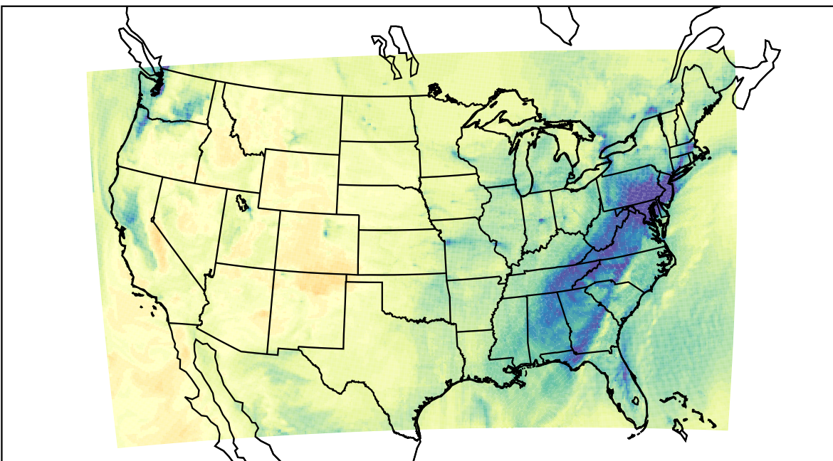
WRF (2019-12-17_21:00:00)
