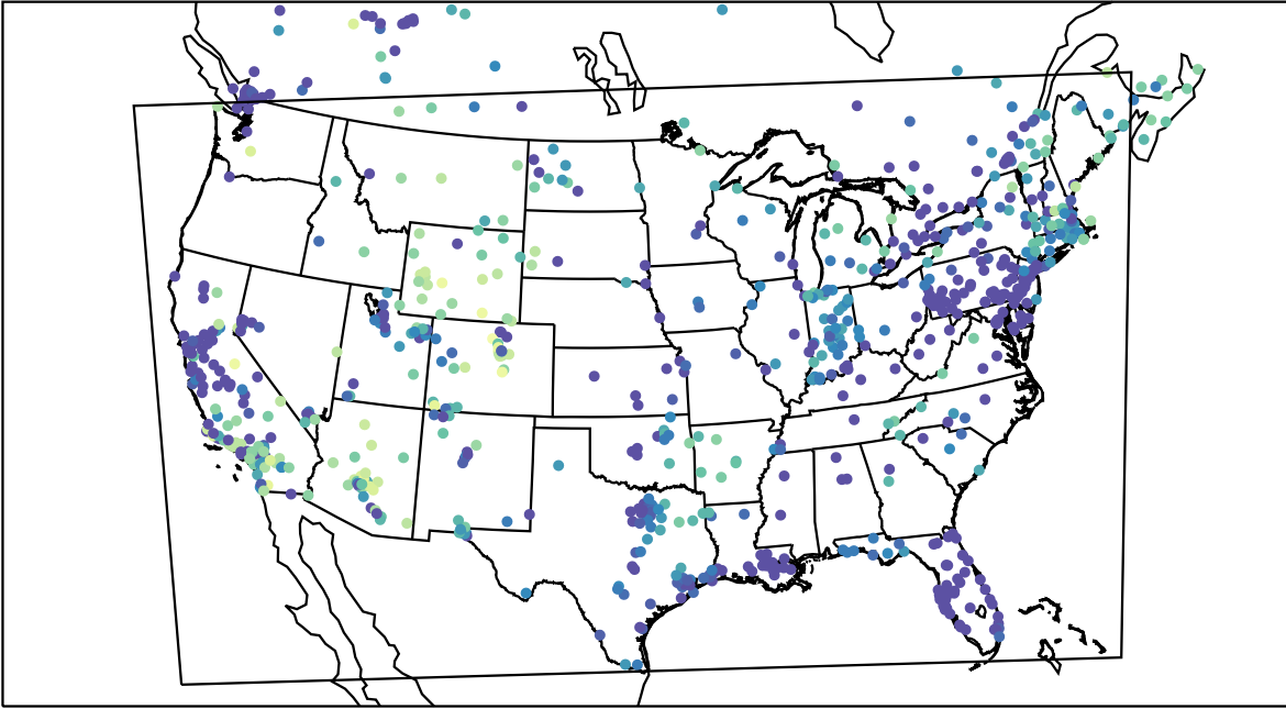
AirNOW (2019-12-17_12:00:00)
