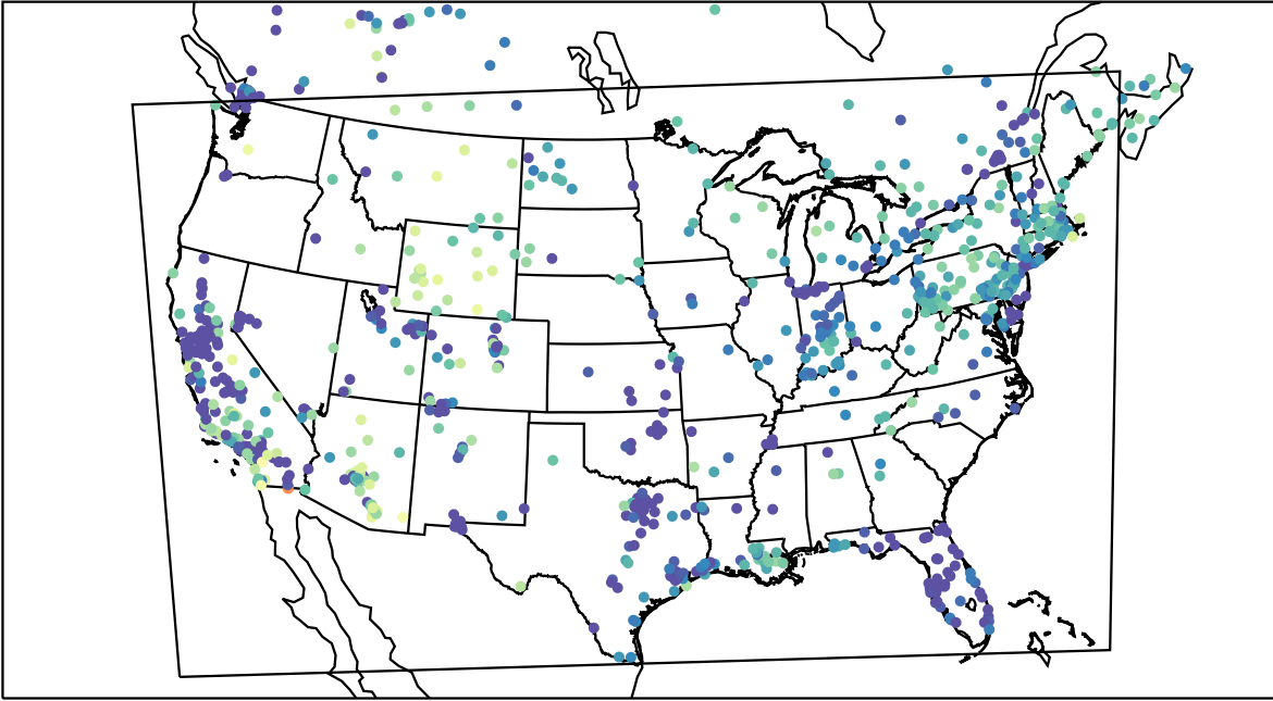
AirNOW (2019-12-18_04:00:00)
