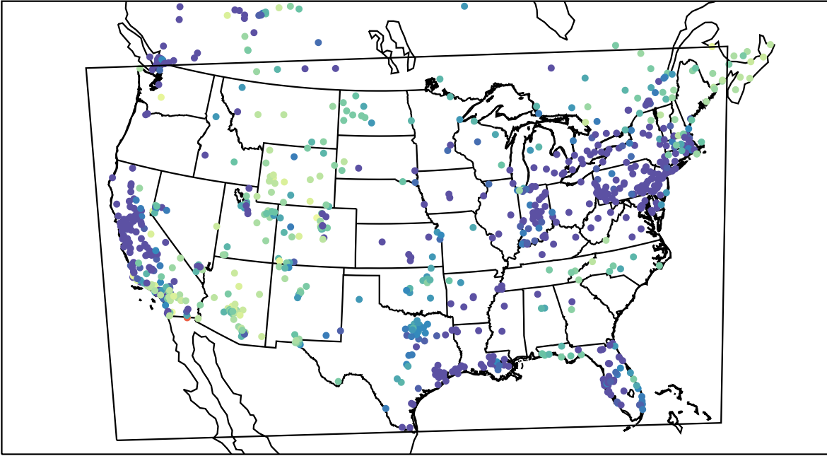
AirNOW (2019-12-17_04:00:00)
