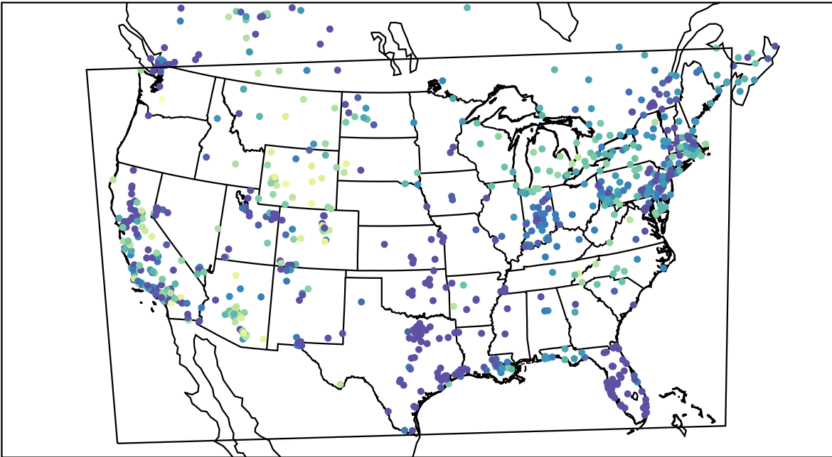
AirNOW (2019-12-18_11:00:00)
