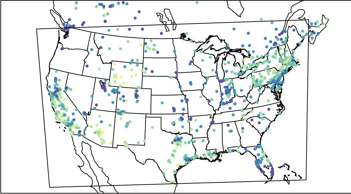
AirNOW (2019-12-18_23:00:00)
