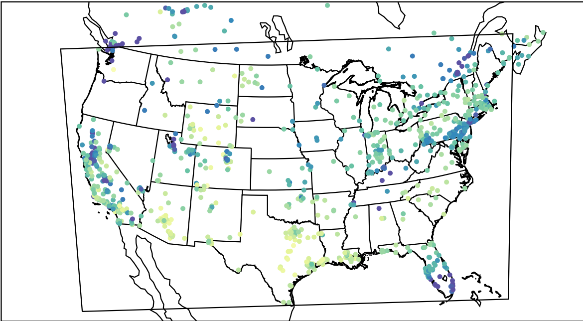
AirNOW (2019-12-18_20:00:00)
