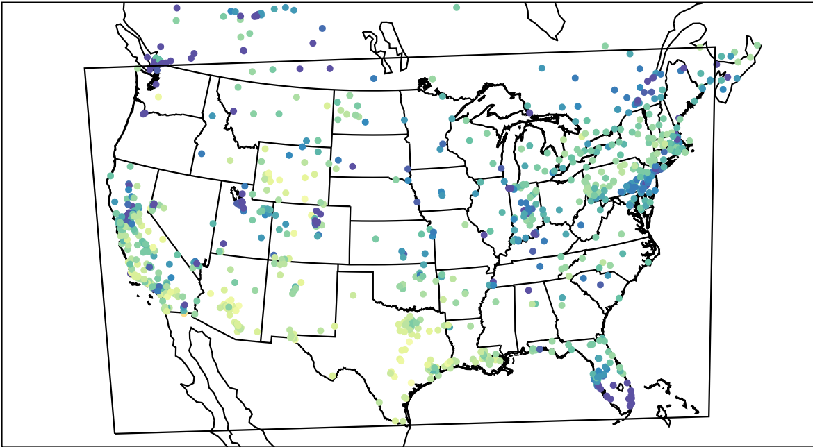
AirNOW (2019-12-18_22:00:00)
