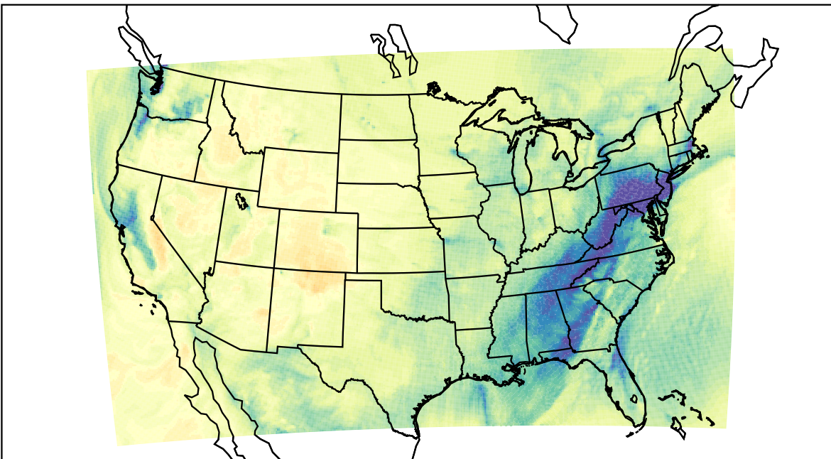
WRF (2019-12-17_19:00:00)
