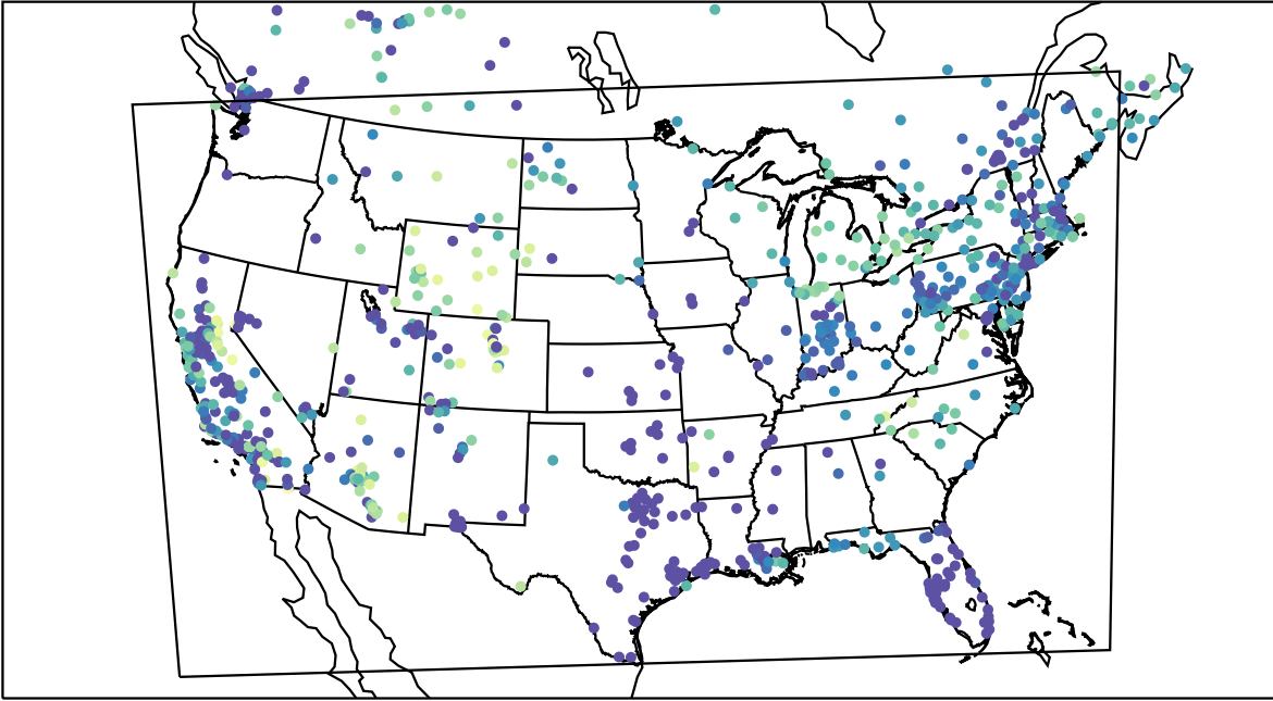
AirNOW (2019-12-18_13:00:00)
