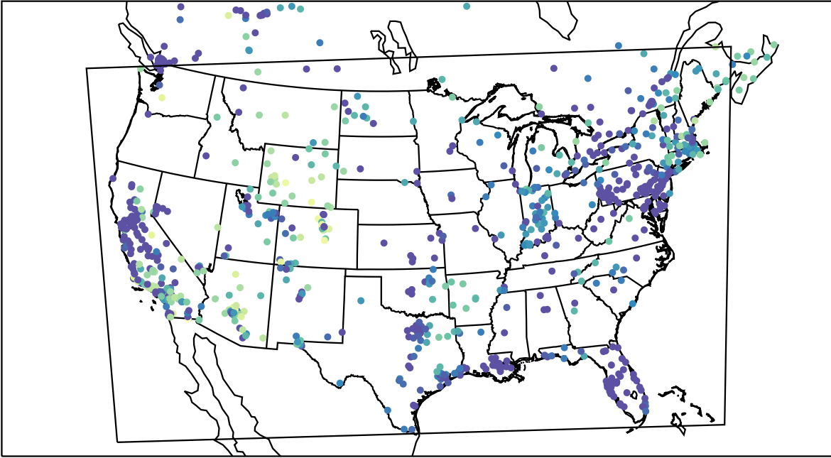
AirNOW (2019-12-17_13:00:00)
