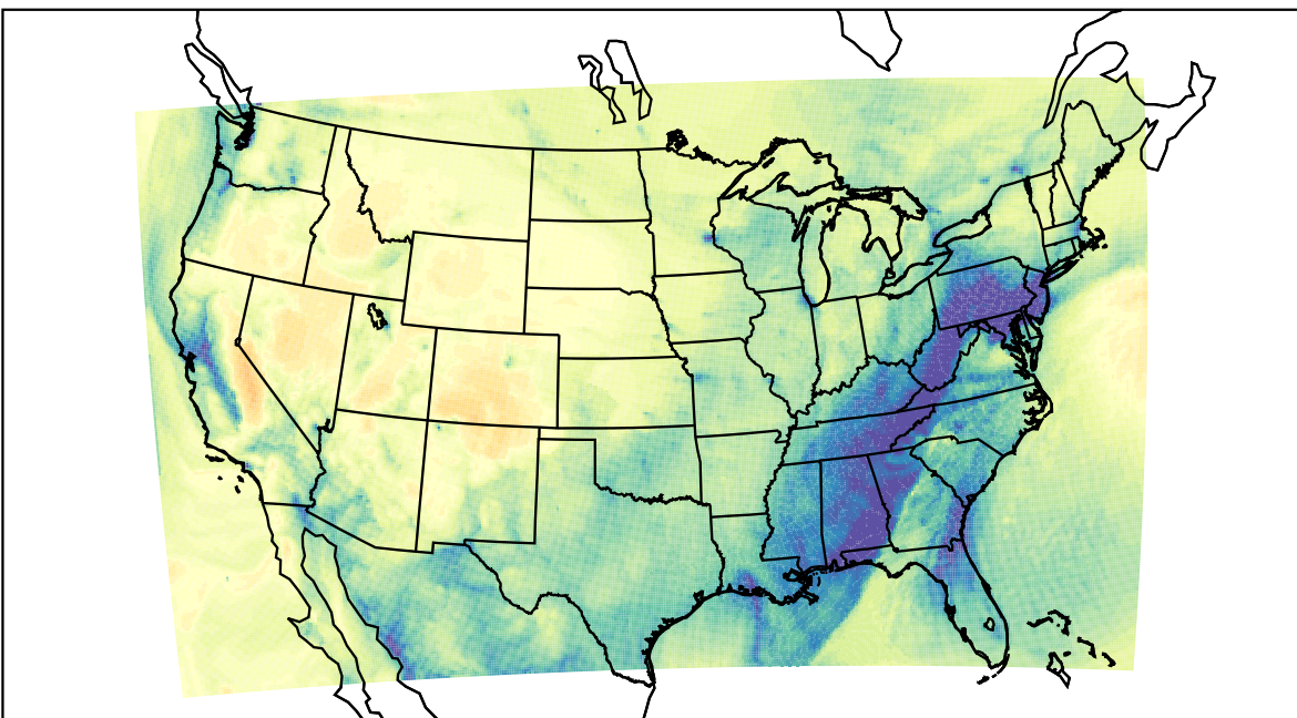
WRF (2019-12-17_16:00:00)
