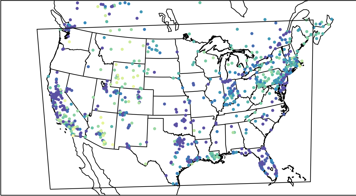
AirNOW (2019-12-18_03:00:00)
