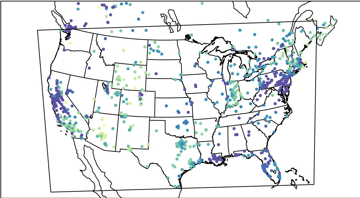
AirNOW (2019-12-17_17:00:00)
