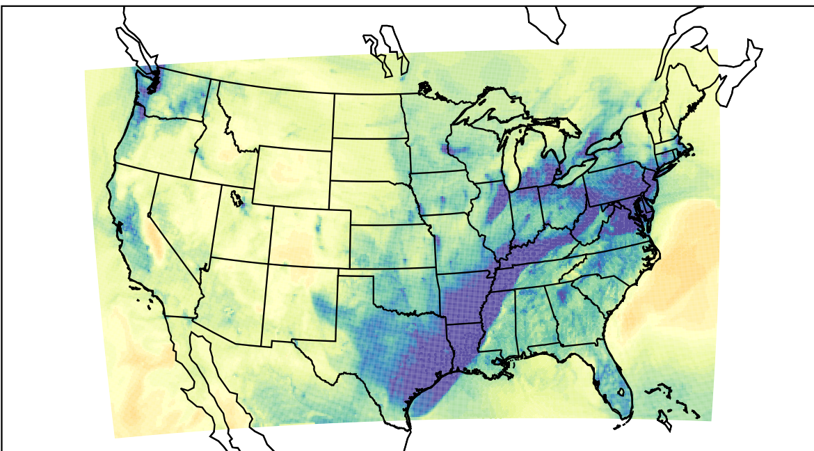
WRF (2019-12-17_00:00:00)
