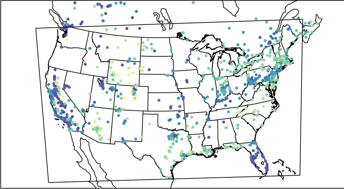
AirNOW (2019-12-18_17:00:00)
