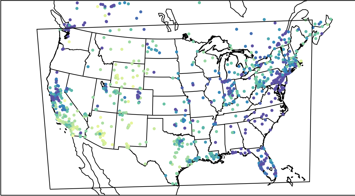
AirNOW (2019-12-17_23:00:00)
