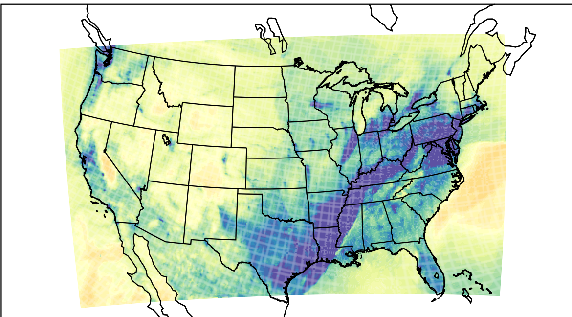
WRF (2019-12-17_02:00:00)
