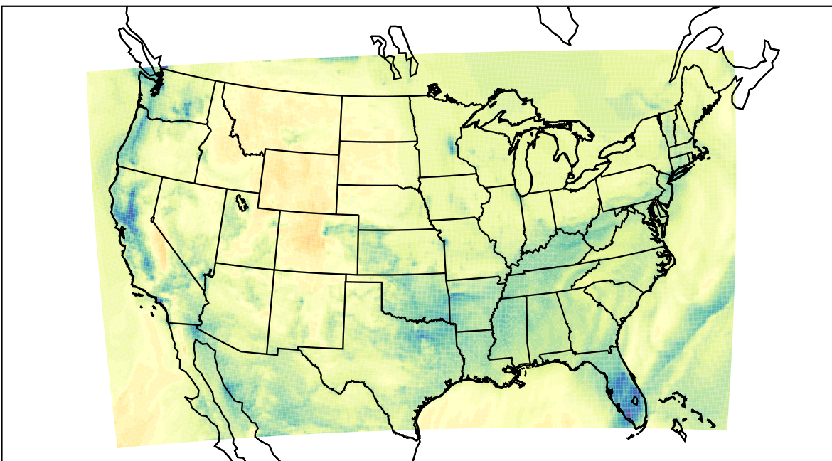
WRF (2019-12-18_18:00:00)
