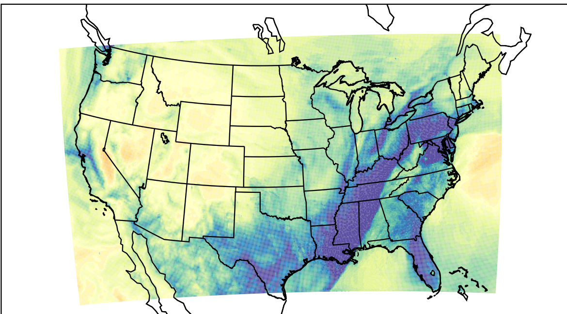
WRF (2019-12-17_09:00:00)
