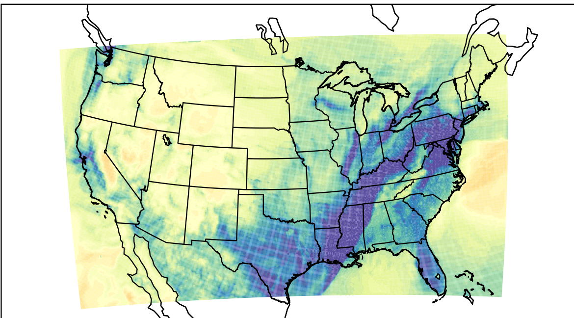
WRF (2019-12-17_06:00:00)
