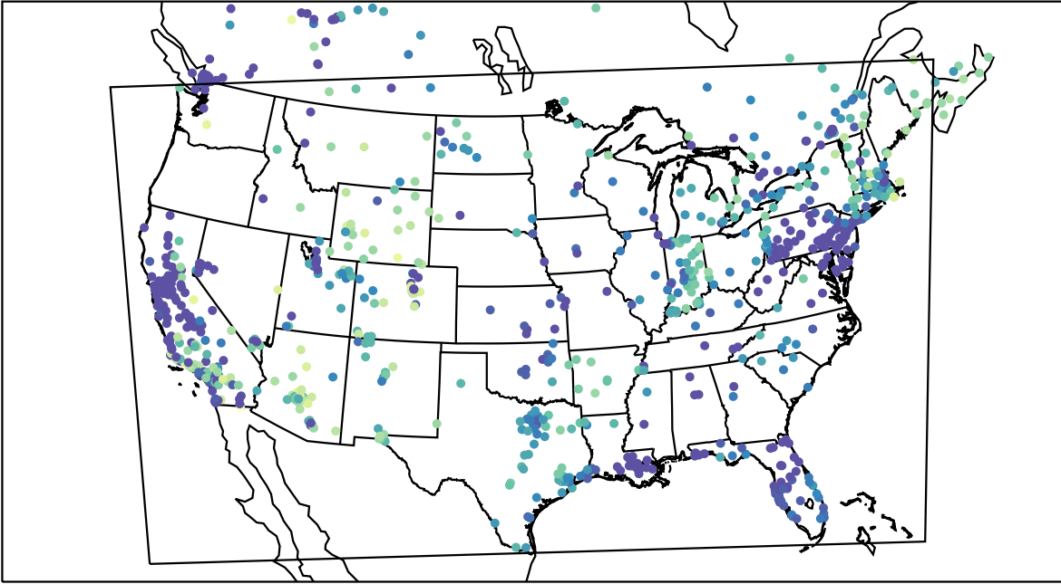
AirNOW (2019-12-17_16:00:00)
