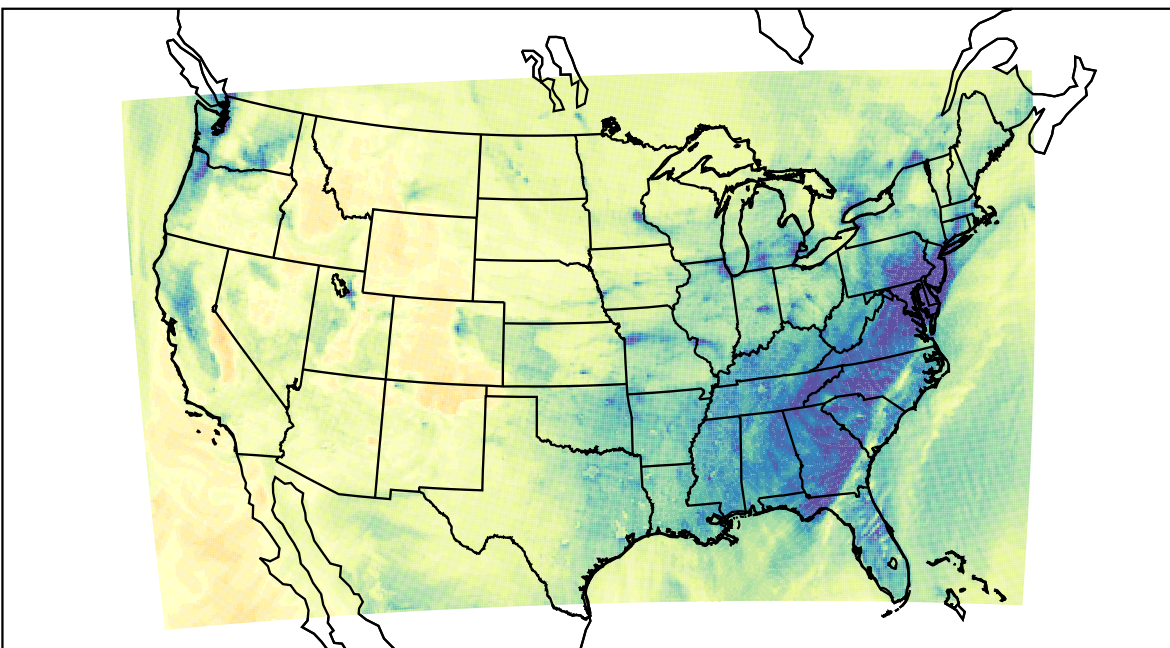
WRF (2019-12-17_23:00:00)
