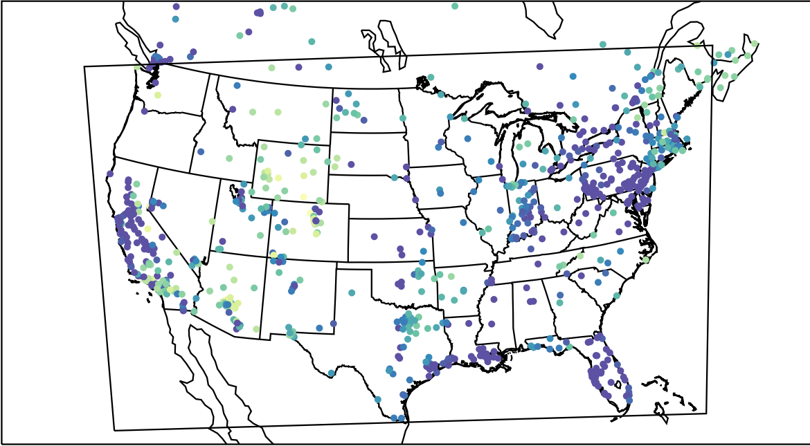
AirNOW (2019-12-17_10:00:00)
