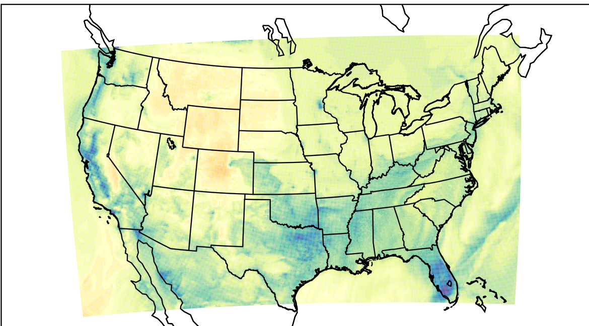
WRF (2019-12-18_17:00:00)
