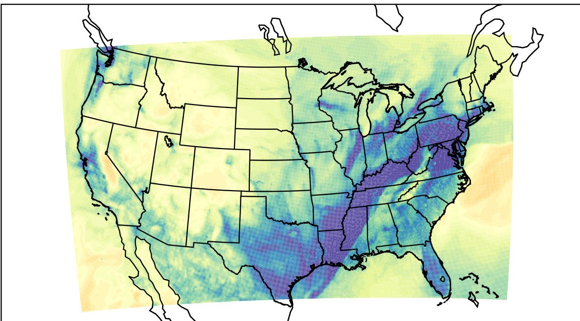
WRF (2019-12-17_04:00:00)
