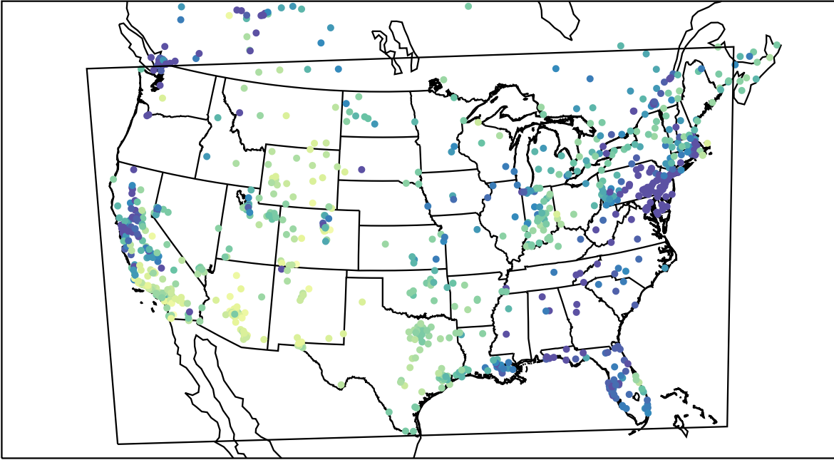
AirNOW (2019-12-17_20:00:00)
