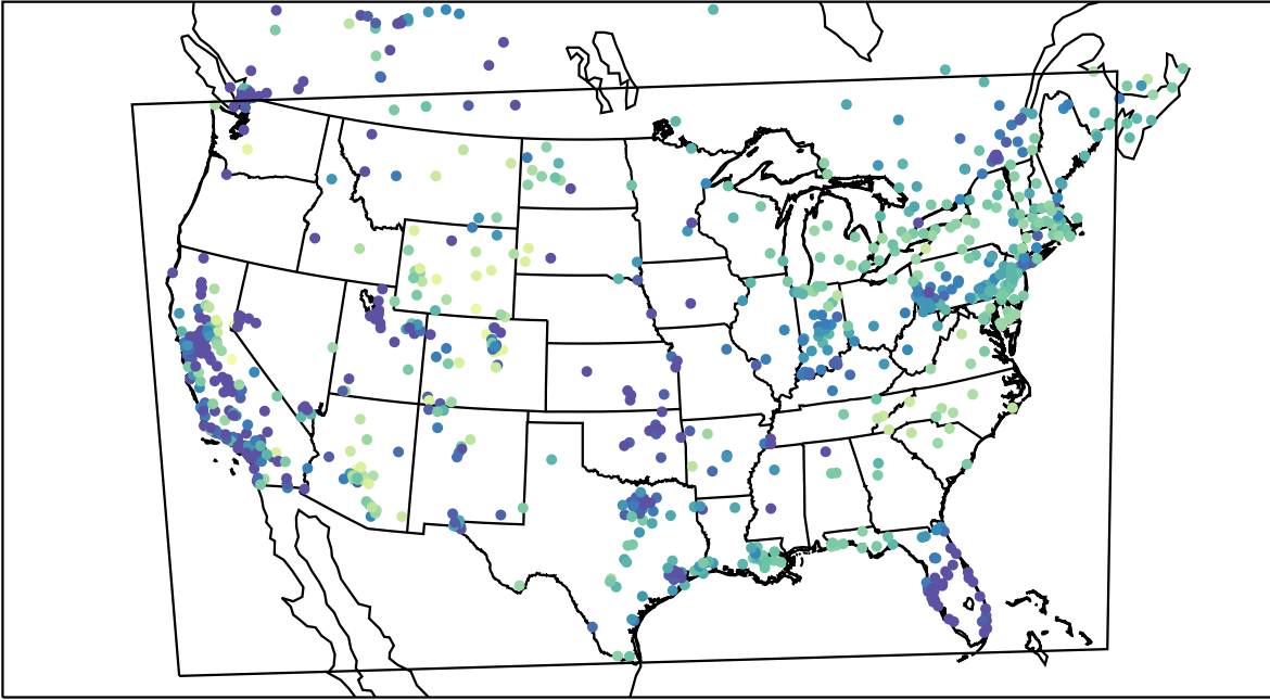
AirNOW (2019-12-18_16:00:00)
