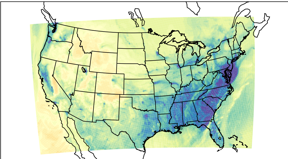
WRF (2019-12-18_01:00:00)
