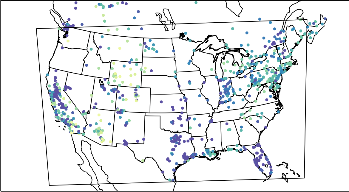
AirNOW (2019-12-18_08:00:00)
