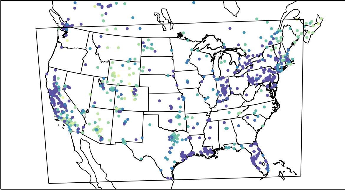
AirNOW (2019-12-17_07:00:00)
