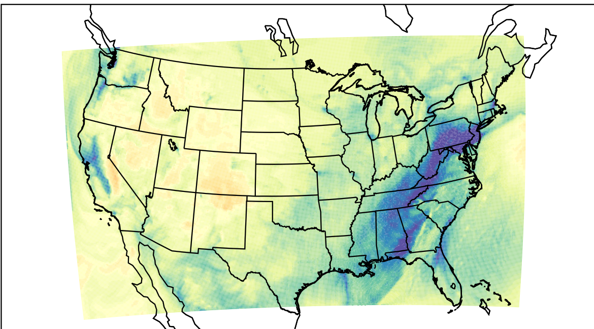
WRF (2019-12-17_18:00:00)
