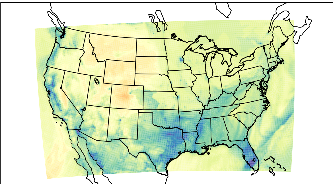
WRF (2019-12-18_16:00:00)
