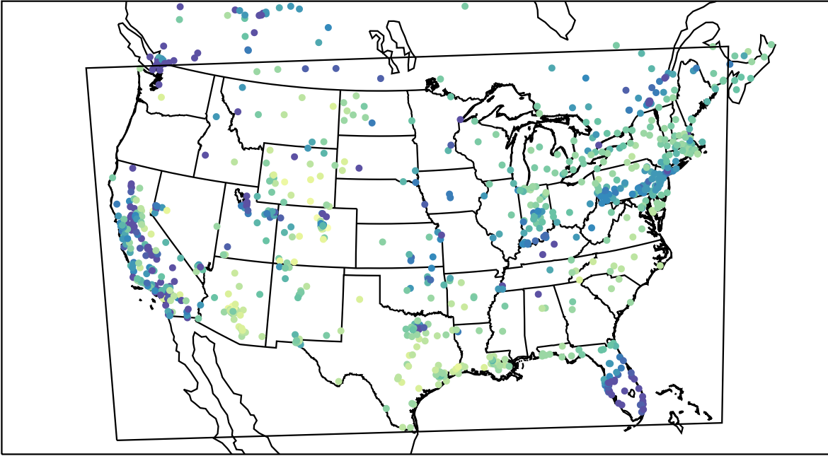
AirNOW (2019-12-18_18:00:00)
