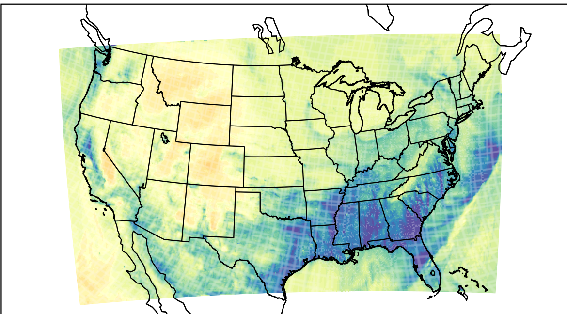
WRF (2019-12-18_09:00:00)
