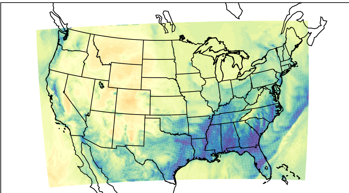
WRF (2019-12-18_11:00:00)
