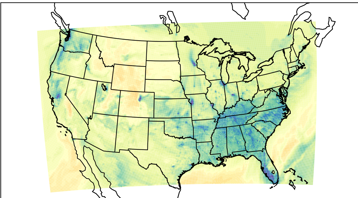
WRF (2019-12-18_23:00:00)
