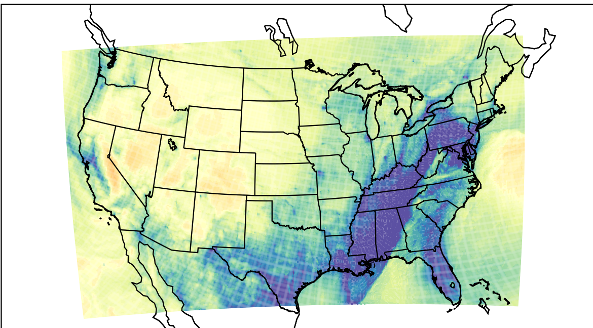
WRF (2019-12-17_13:00:00)
