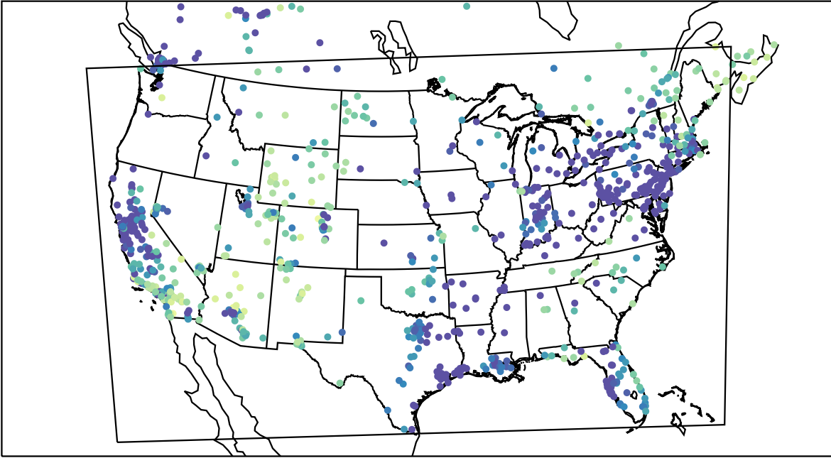
AirNOW (2019-12-17_01:00:00)
