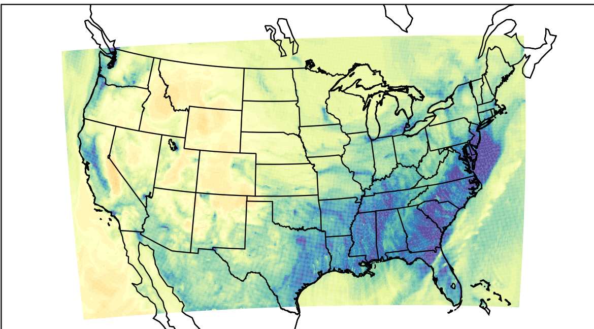
WRF (2019-12-18_03:00:00)
