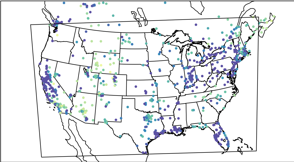
AirNOW (2019-12-17_06:00:00)
