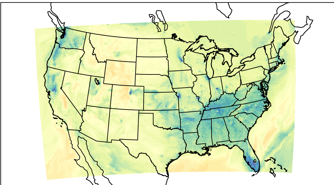
WRF (2019-12-18_22:00:00)
