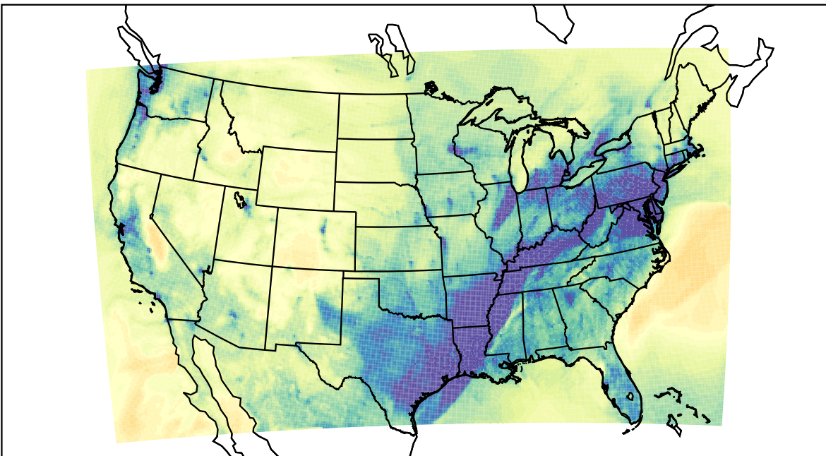
WRF (2019-12-17_01:00:00)
