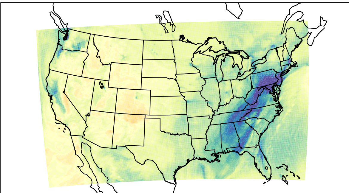
WRF (2019-12-17_20:00:00)
