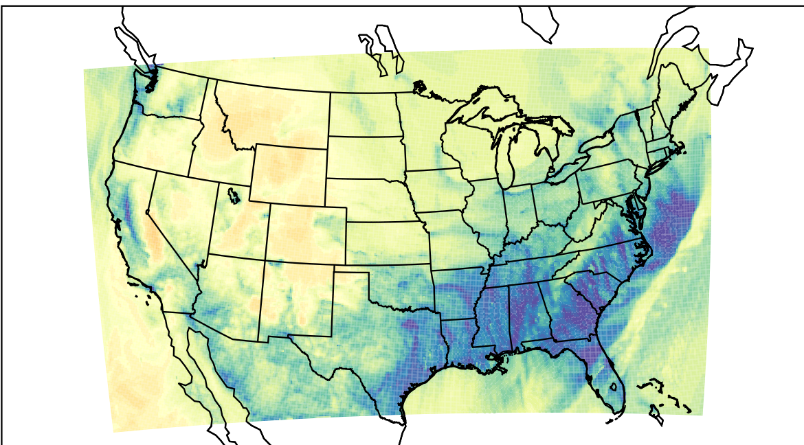
WRF (2019-12-18_06:00:00)
