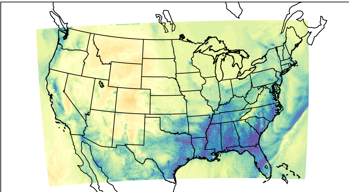
WRF (2019-12-18_12:00:00)
