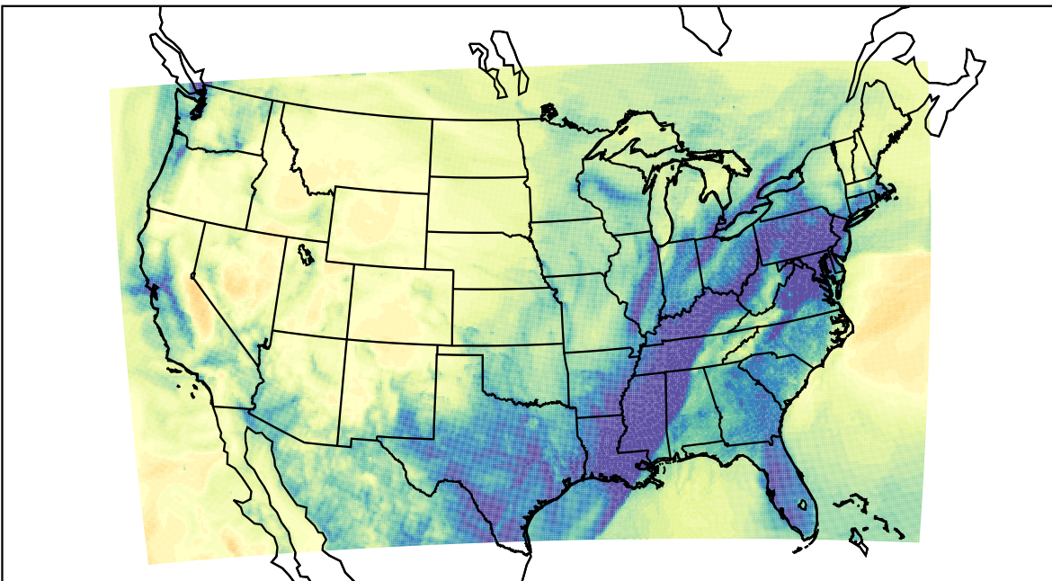
WRF (2019-12-17_07:00:00)
