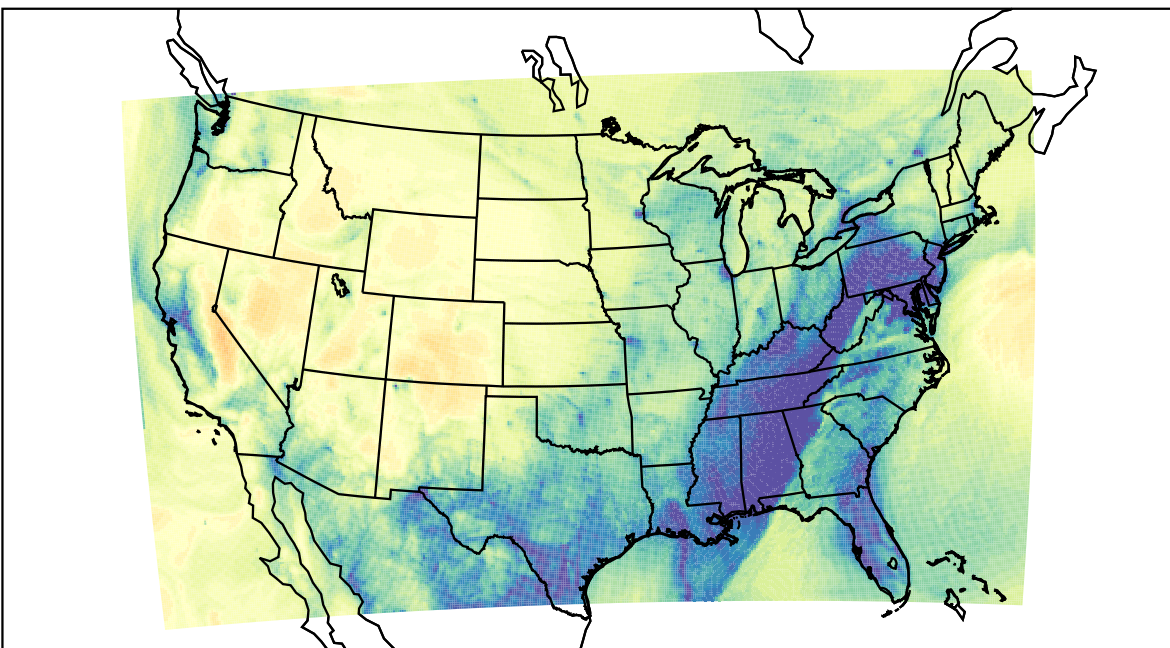
WRF (2019-12-17_14:00:00)
