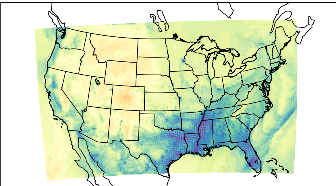
WRF (2019-12-18_14:00:00)
