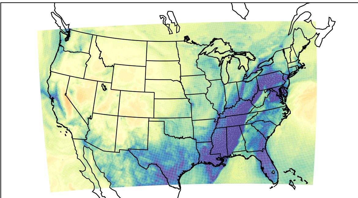
WRF (2019-12-17_11:00:00)
