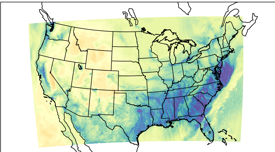
WRF (2019-12-18_04:00:00)
