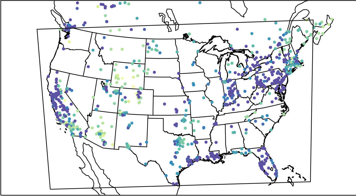
AirNOW (2019-12-17_08:00:00)
