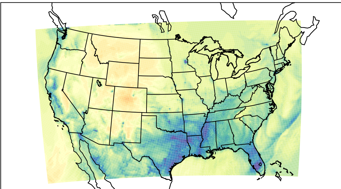
WRF (2019-12-18_15:00:00)
