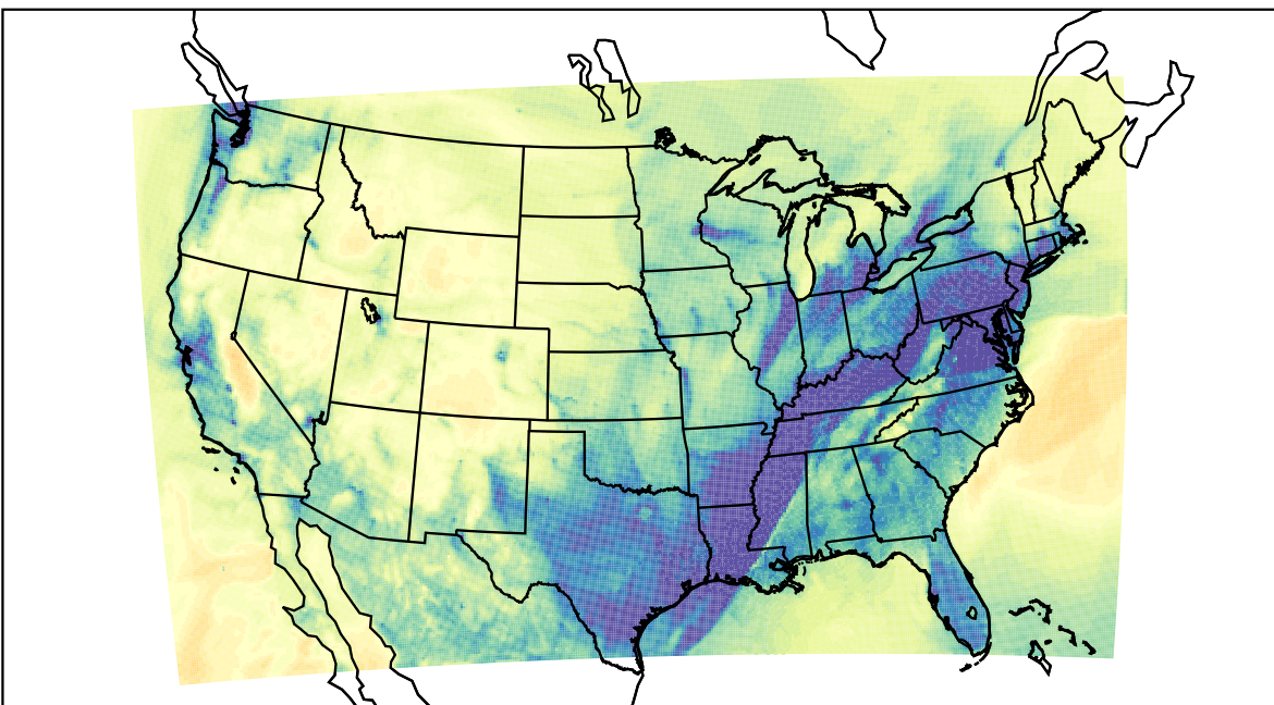
WRF (2019-12-17_03:00:00)
