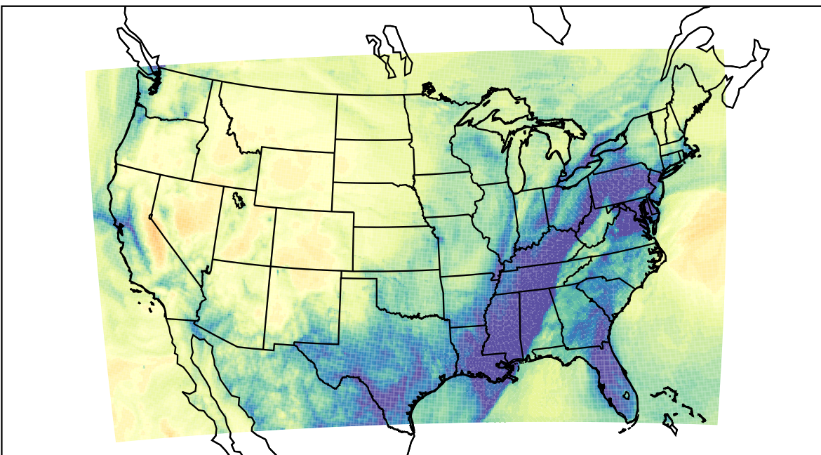
WRF (2019-12-17_10:00:00)
