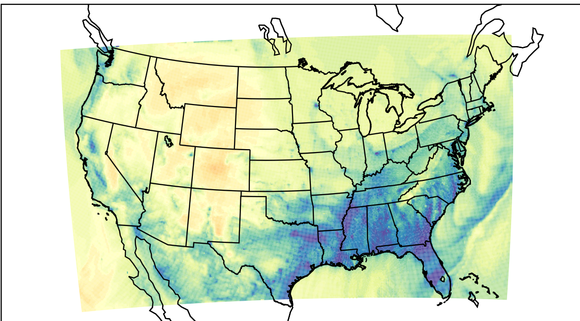
WRF (2019-12-18_13:00:00)
