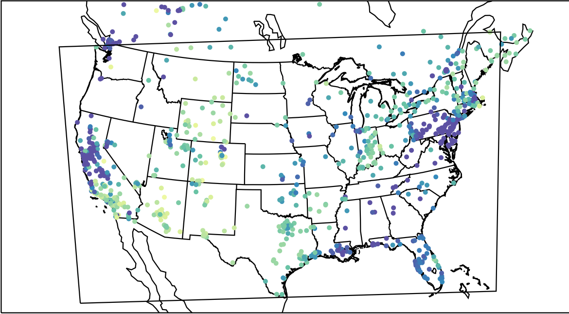
AirNOW (2019-12-17_18:00:00)
