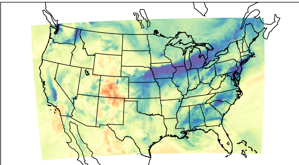
WRF (2019-12-23_20:00:00)
