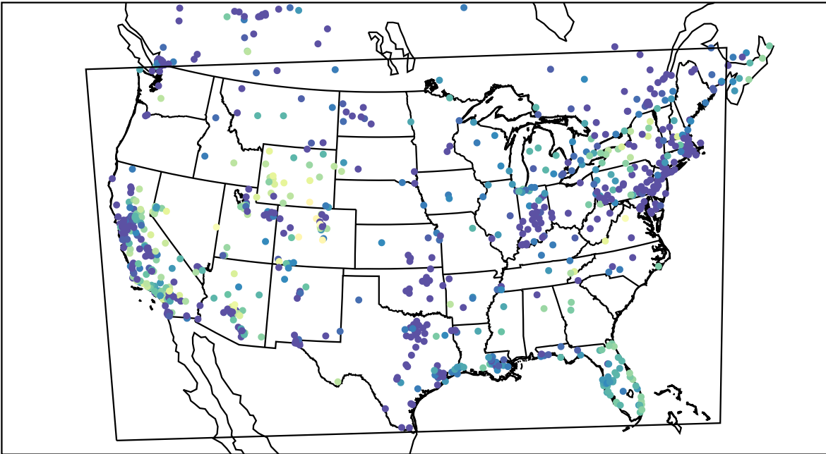
AirNOW (2019-12-23_04:00:00)
