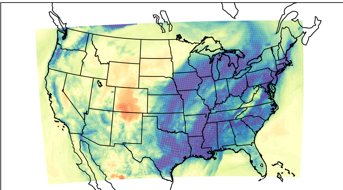
WRF (2019-12-22_10:00:00)
