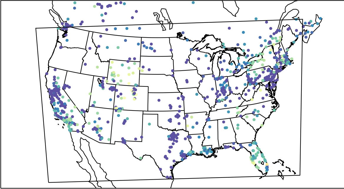
AirNOW (2019-12-23_15:00:00)
