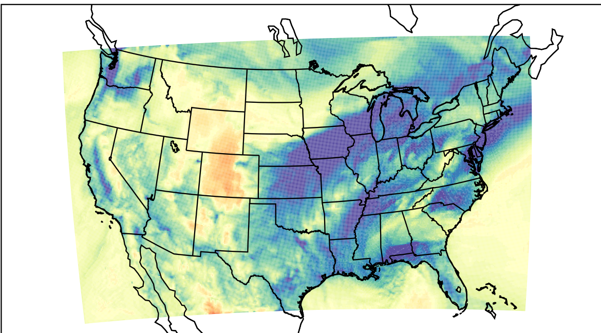
WRF (2019-12-23_08:00:00)
