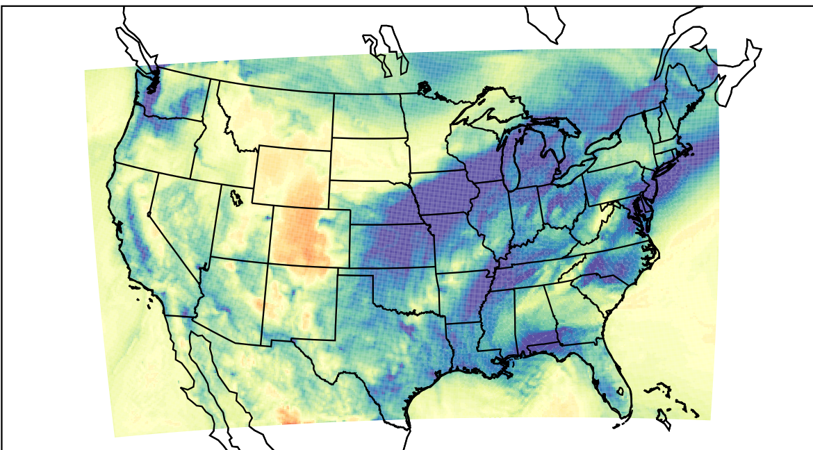
WRF (2019-12-23_07:00:00)
