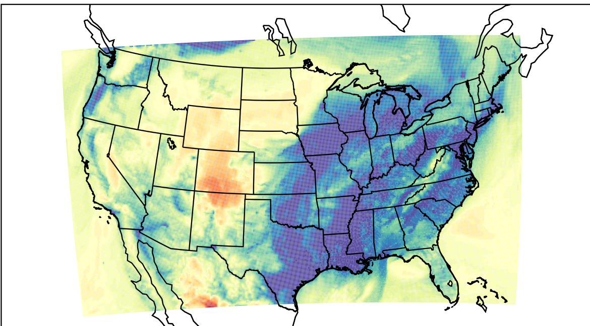
WRF (2019-12-22_14:00:00)
