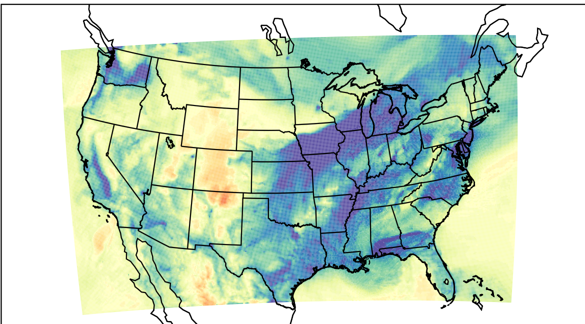
WRF (2019-12-23_14:00:00)
