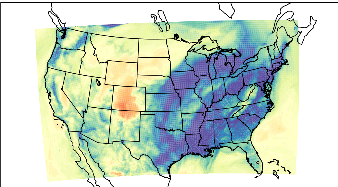
WRF (2019-12-22_08:00:00)
