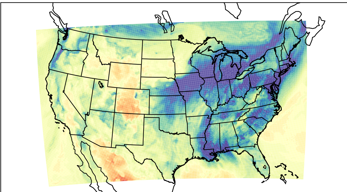
WRF (2019-12-22_22:00:00)
