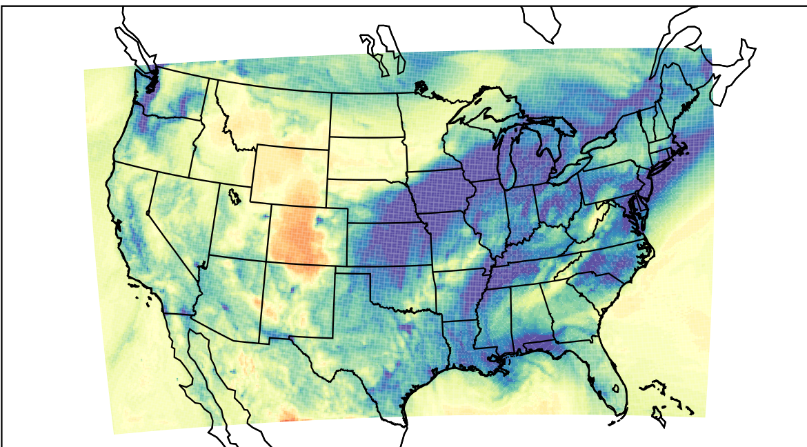
WRF (2019-12-23_04:00:00)
