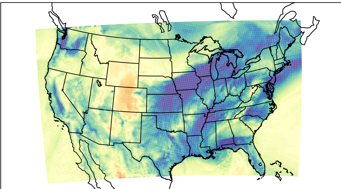
WRF (2019-12-23_09:00:00)
