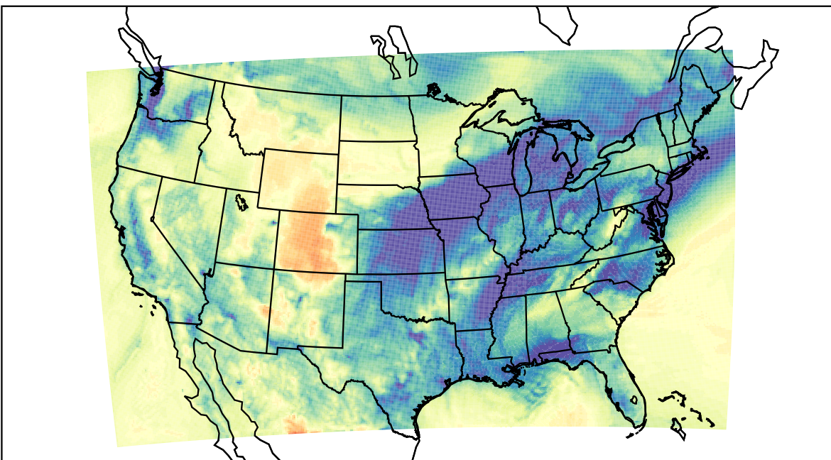
WRF (2019-12-23_06:00:00)
