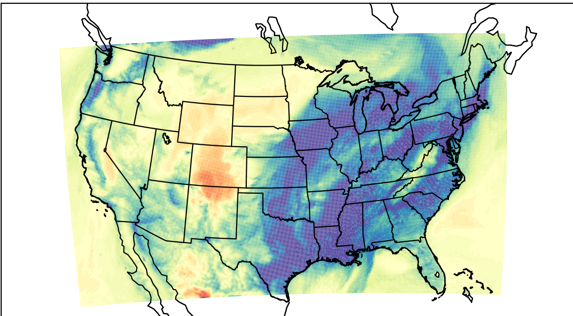
WRF (2019-12-22_12:00:00)
