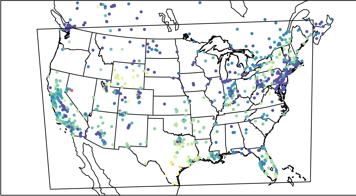
AirNOW (2019-12-23_22:00:00)
