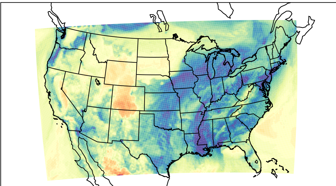
WRF (2019-12-22_17:00:00)
