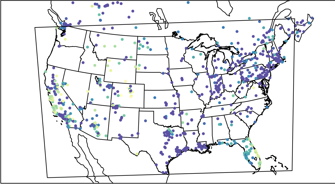
AirNOW (2019-12-22_11:00:00)
