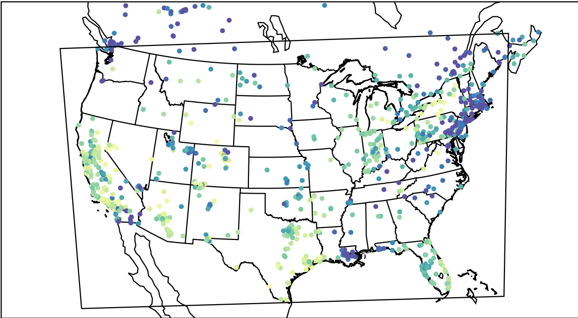
AirNOW (2019-12-22_20:00:00)
