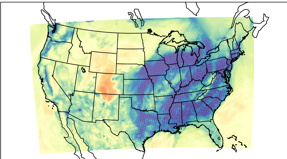
WRF (2019-12-22_03:00:00)
