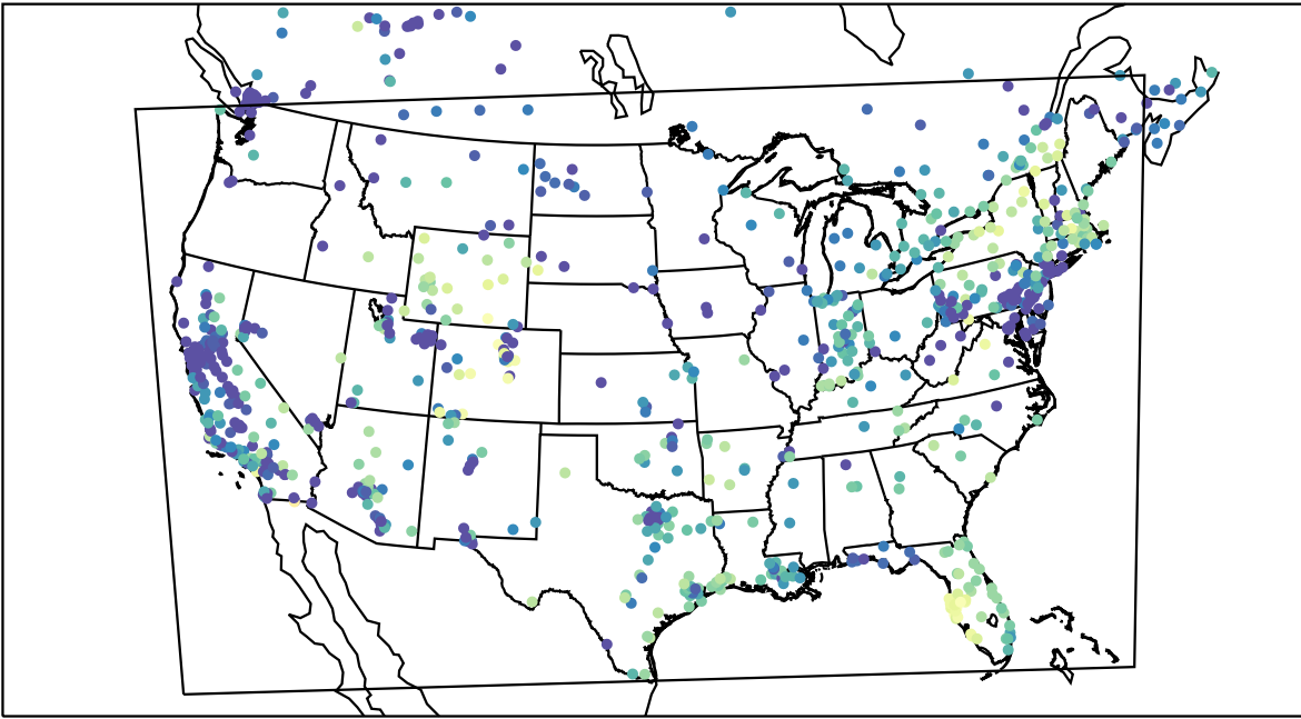
AirNOW (2019-12-23_17:00:00)
