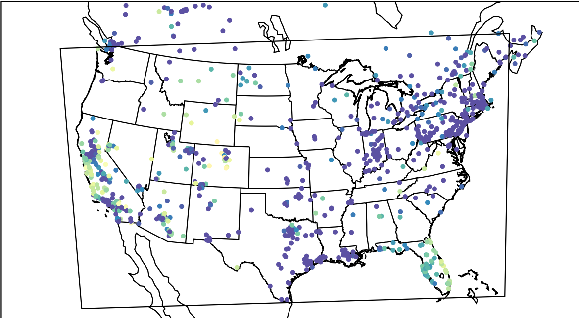
AirNOW (2019-12-22_13:00:00)
