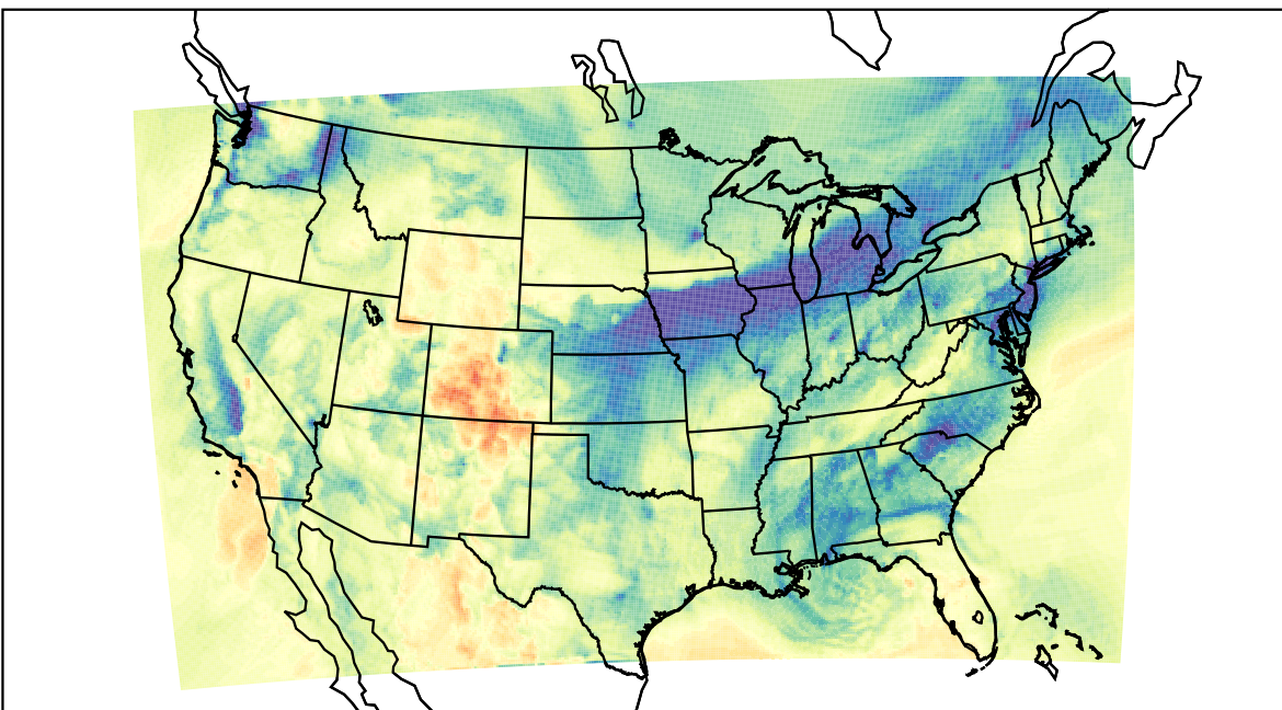
WRF (2019-12-23_19:00:00)
