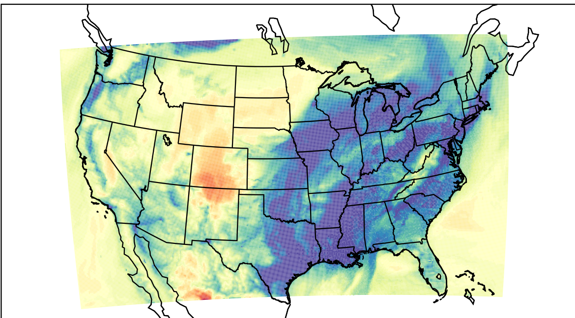
WRF (2019-12-22_13:00:00)
