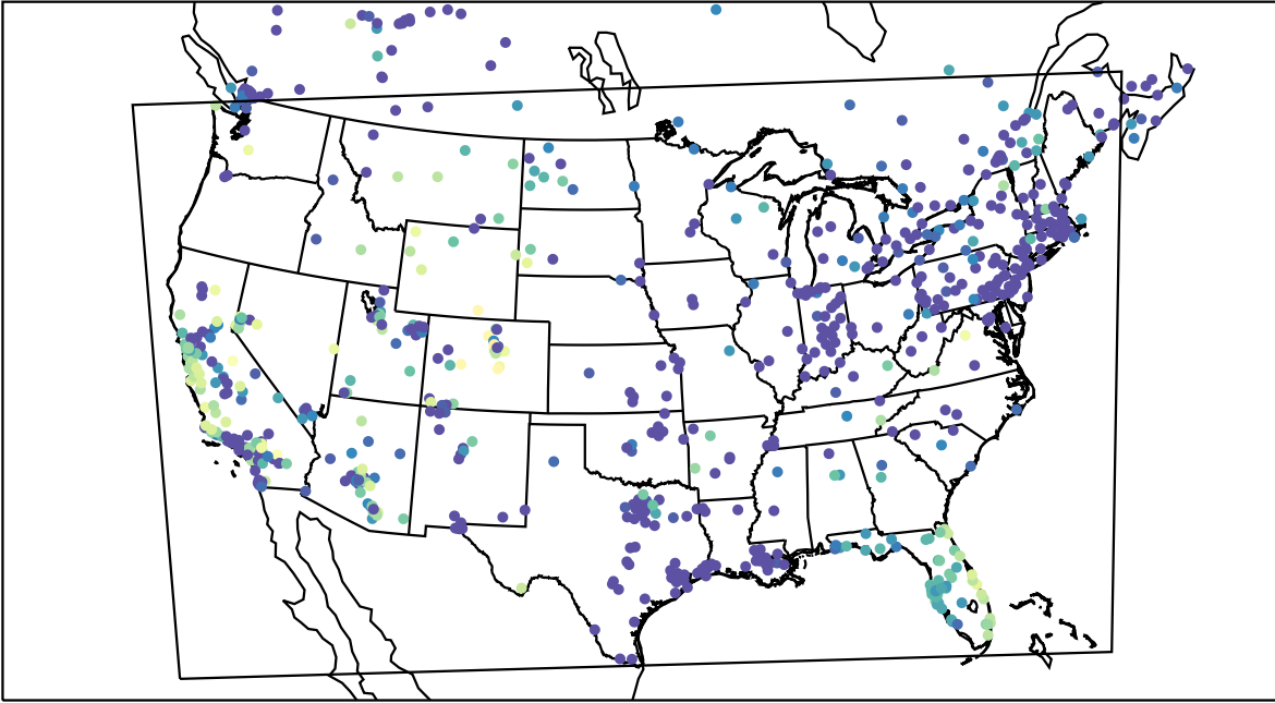
AirNOW (2019-12-22_12:00:00)
