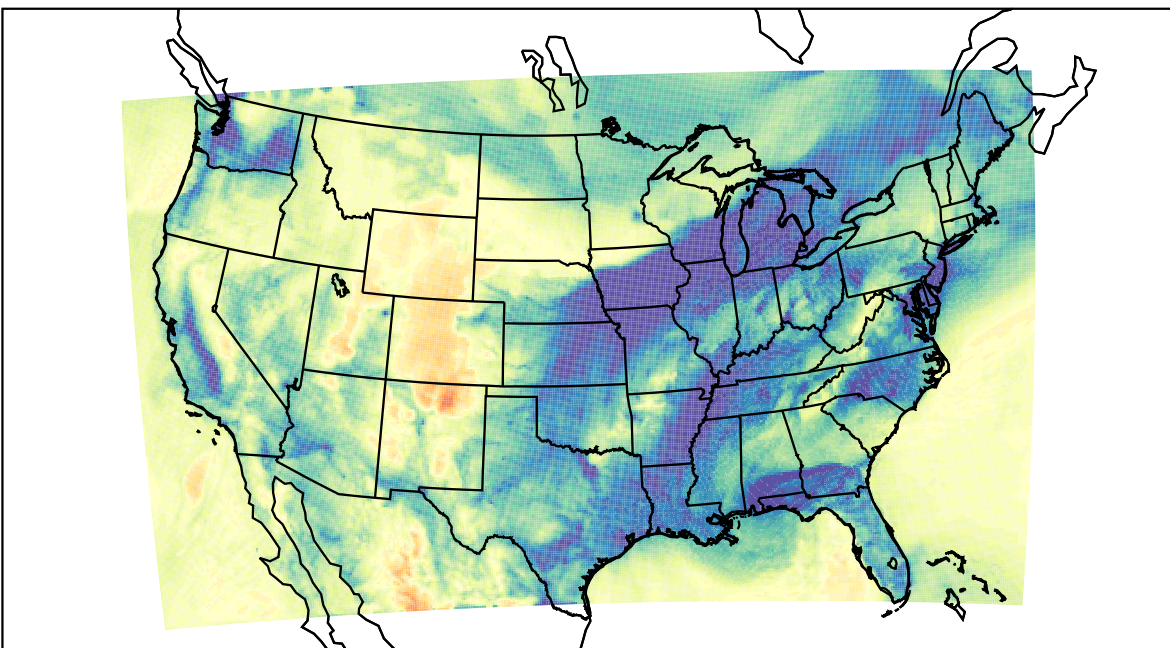
WRF (2019-12-23_13:00:00)
