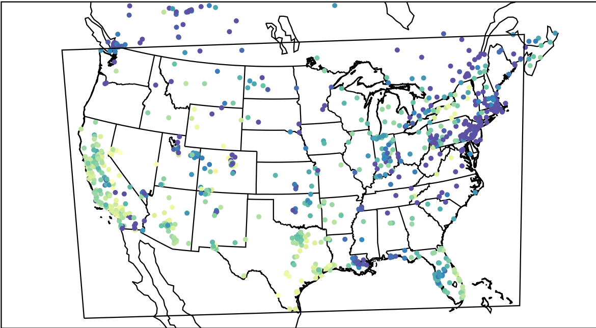
AirNOW (2019-12-22_22:00:00)
