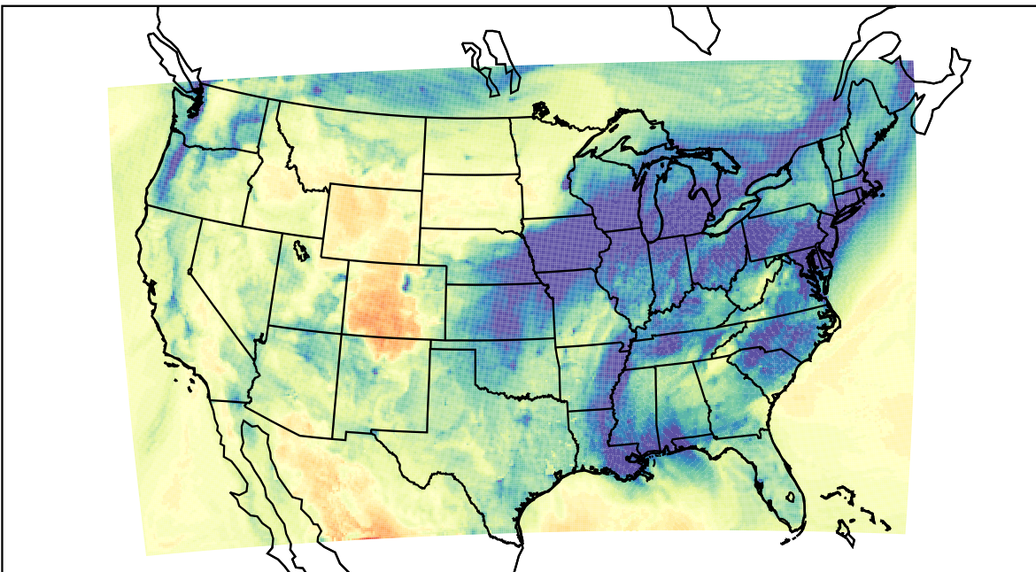
WRF (2019-12-22_23:00:00)
