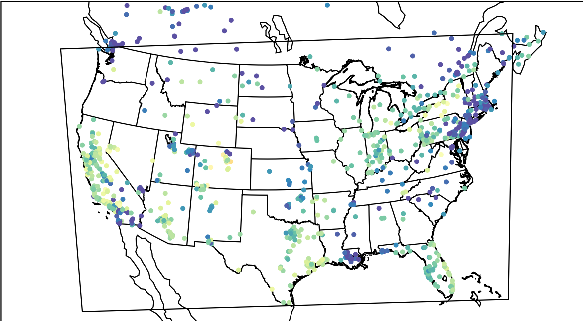
AirNOW (2019-12-22_19:00:00)
