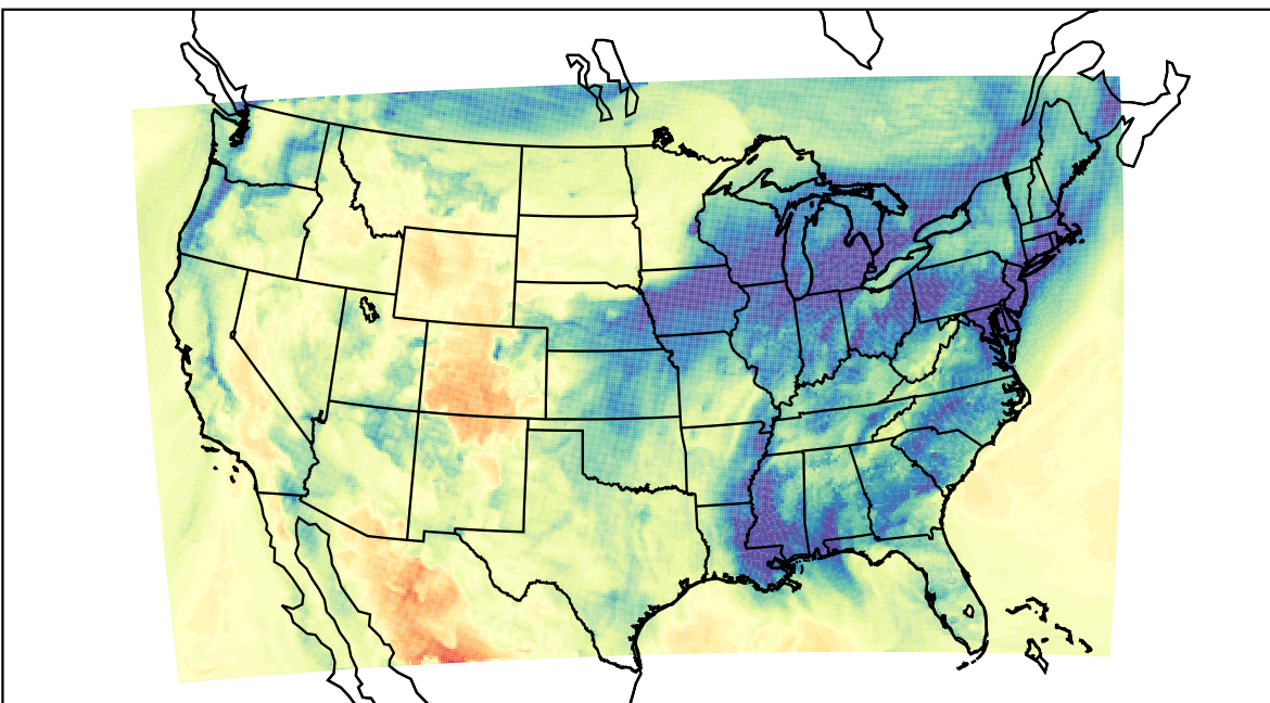
WRF (2019-12-22_21:00:00)
