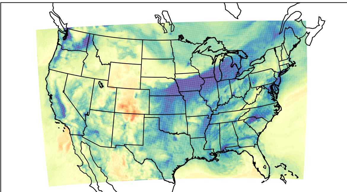
WRF (2019-12-23_17:00:00)
