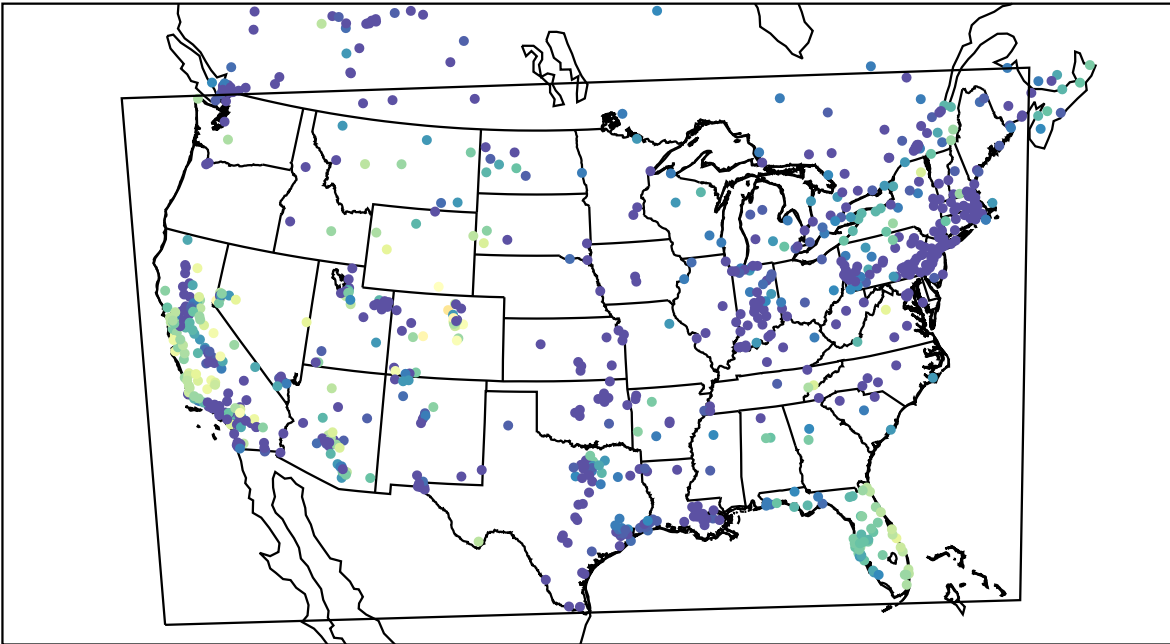
AirNOW (2019-12-22_15:00:00)
