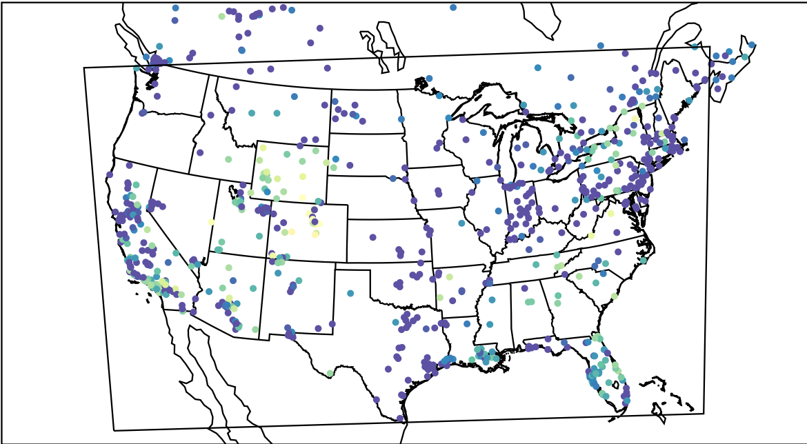
AirNOW (2019-12-23_11:00:00)
