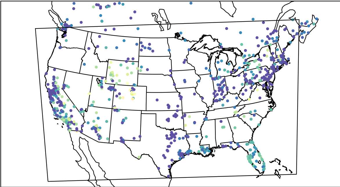
AirNOW (2019-12-23_08:00:00)
