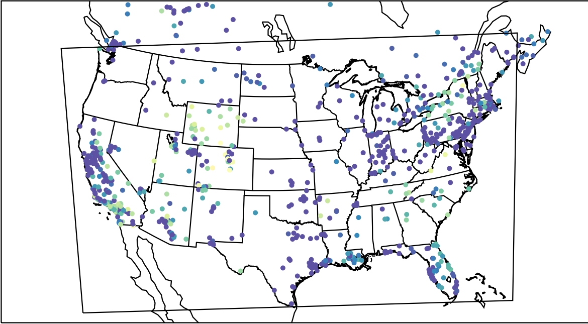
AirNOW (2019-12-23_13:00:00)
