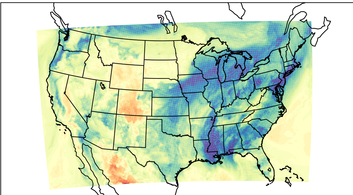
WRF (2019-12-22_19:00:00)
