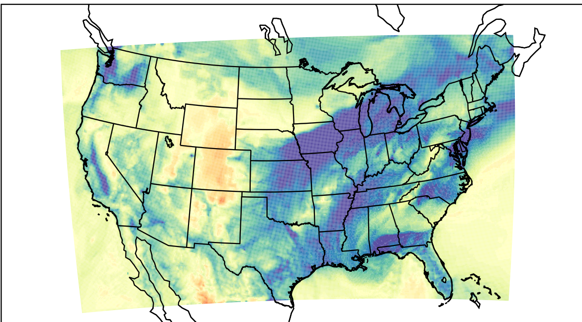
WRF (2019-12-23_11:00:00)
