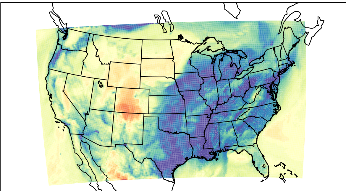
WRF (2019-12-22_15:00:00)
