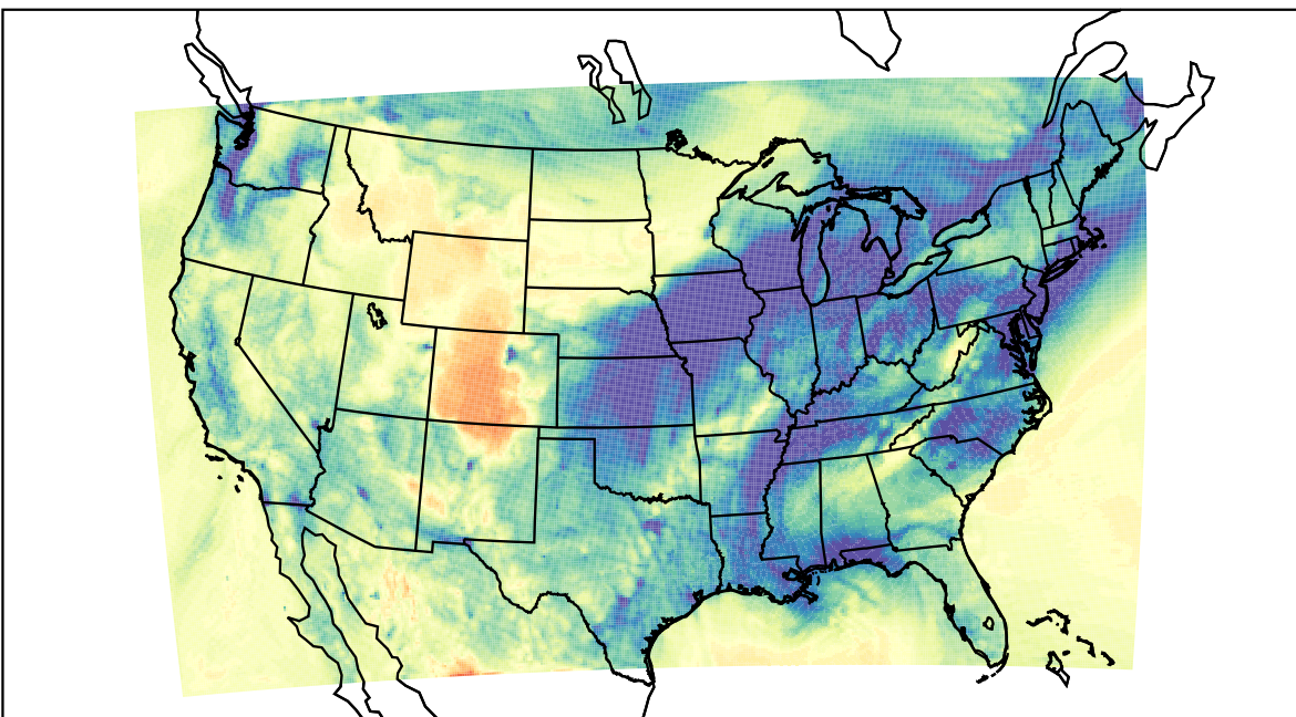
WRF (2019-12-23_03:00:00)
