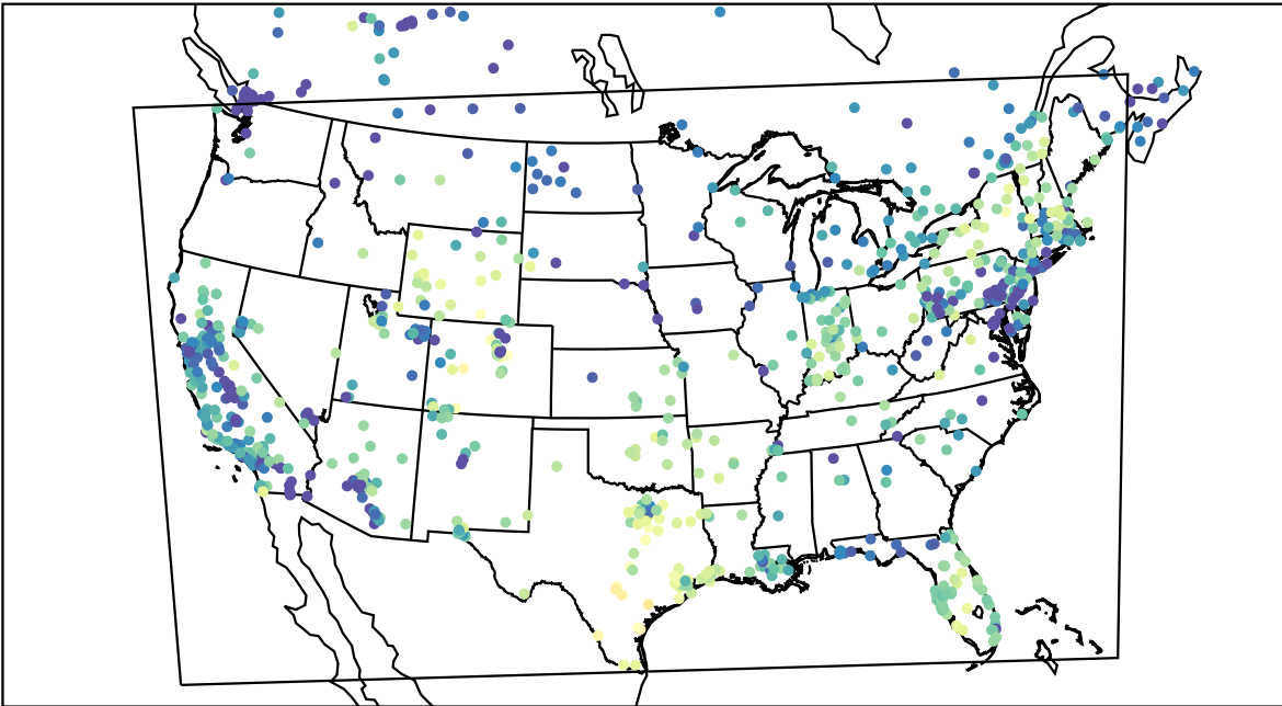
AirNOW (2019-12-23_20:00:00)
