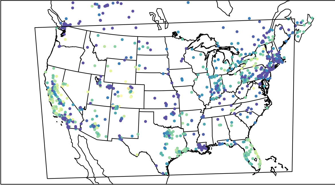
AirNOW (2019-12-22_17:00:00)
