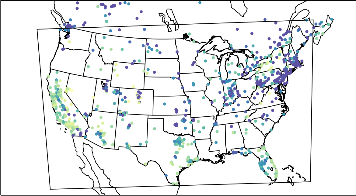
AirNOW (2019-12-22_23:00:00)
