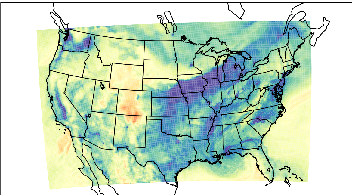
WRF (2019-12-23_16:00:00)
