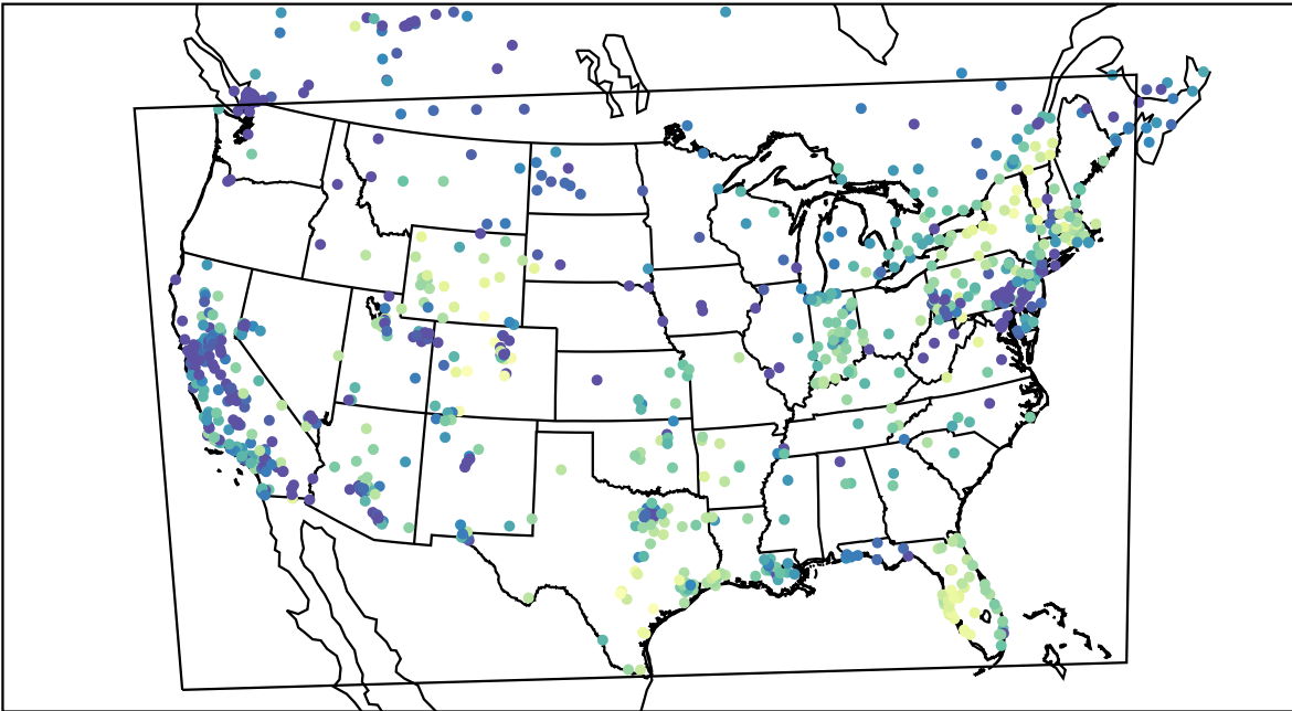
AirNOW (2019-12-23_18:00:00)
