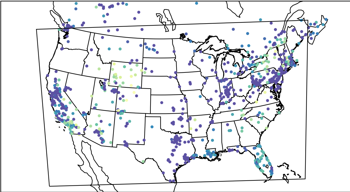
AirNOW (2019-12-23_14:00:00)
