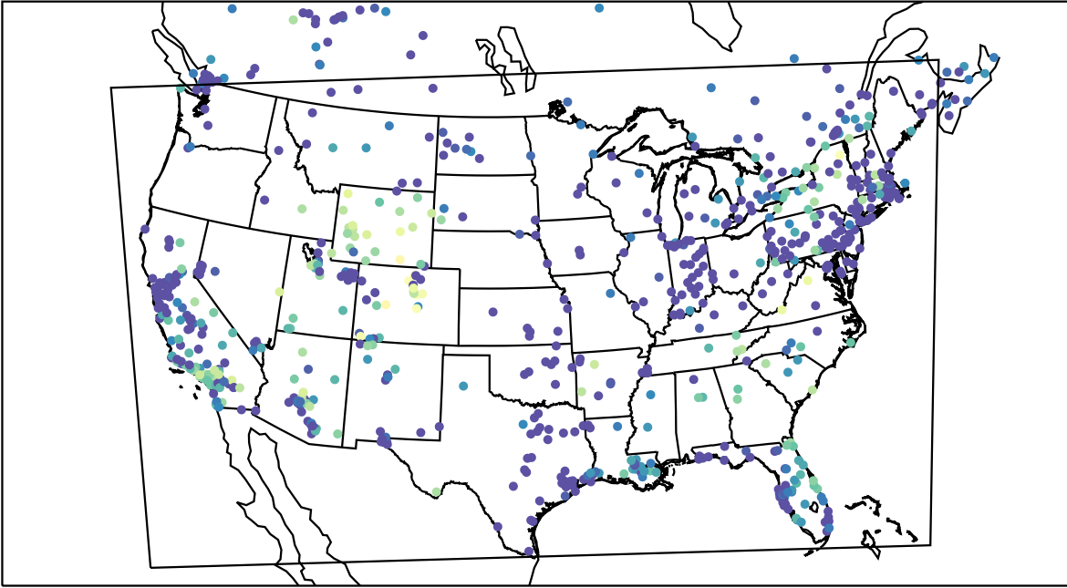
AirNOW (2019-12-23_12:00:00)
