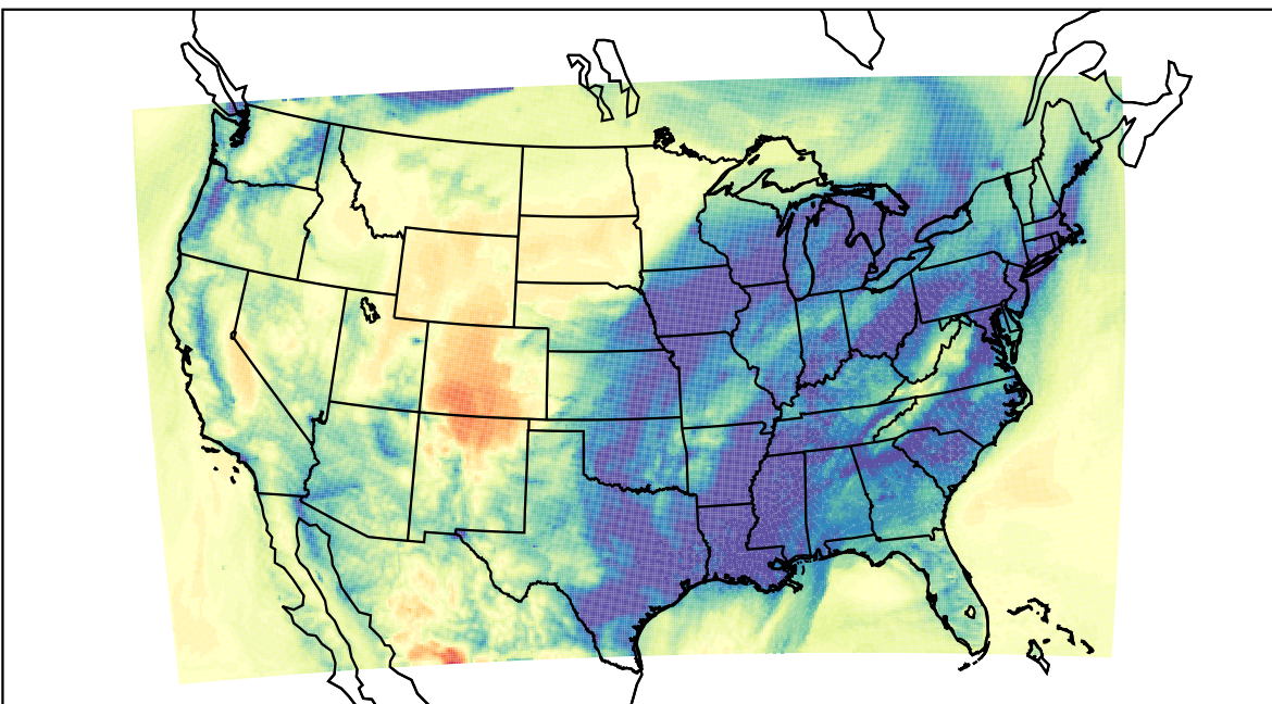
WRF (2019-12-22_11:00:00)
