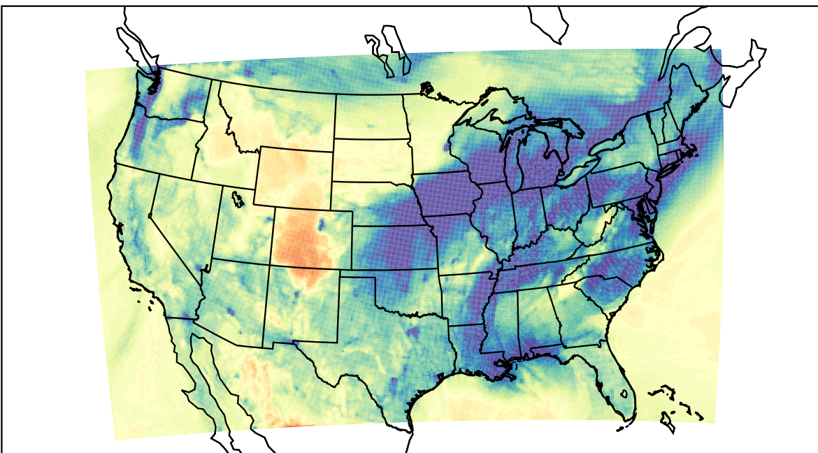
WRF (2019-12-23_01:00:00)
