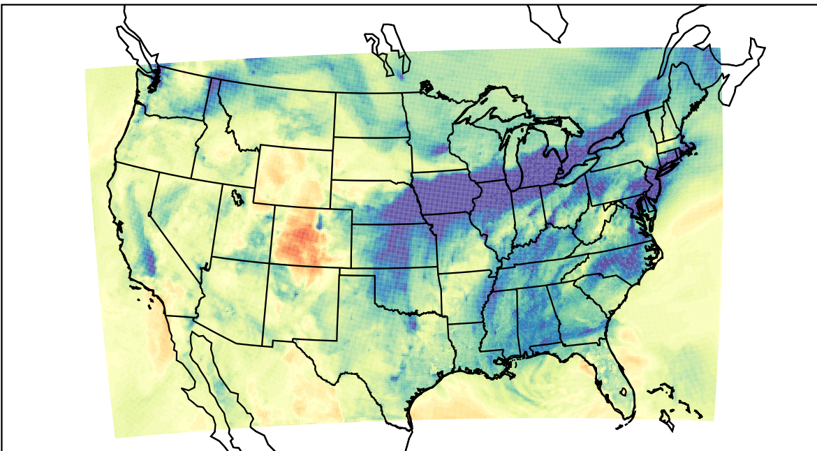
WRF (2019-12-23_23:00:00)
