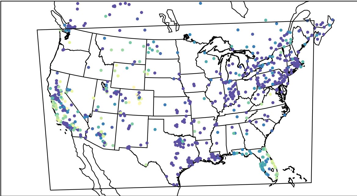
AirNOW (2019-12-22_10:00:00)
