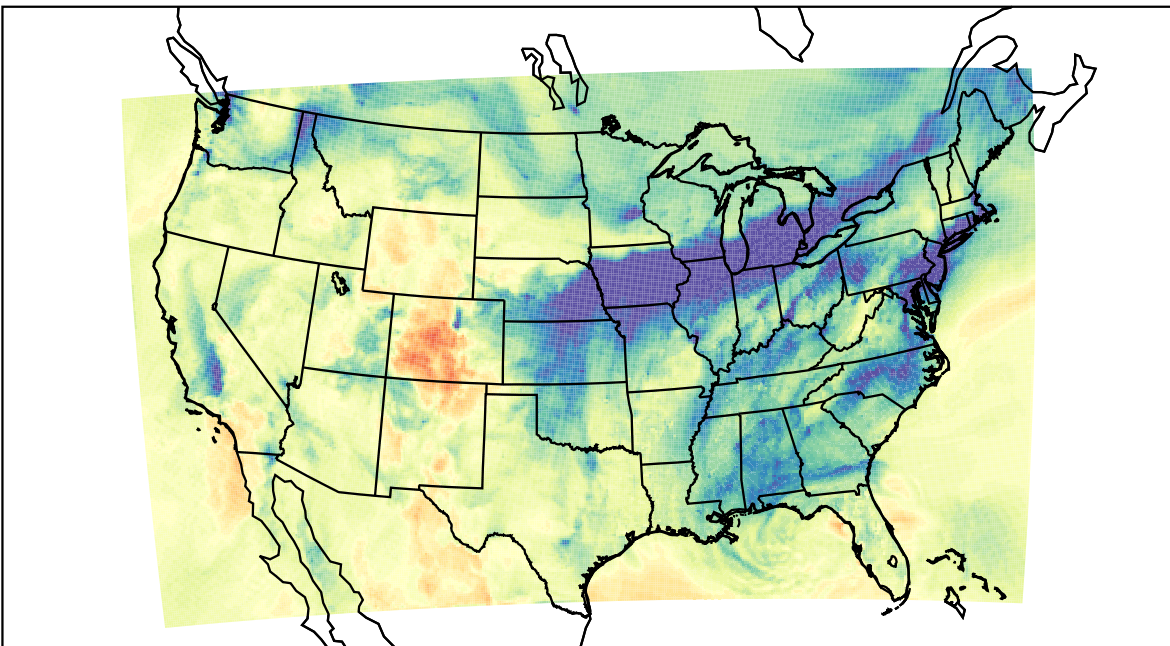
WRF (2019-12-23_22:00:00)
