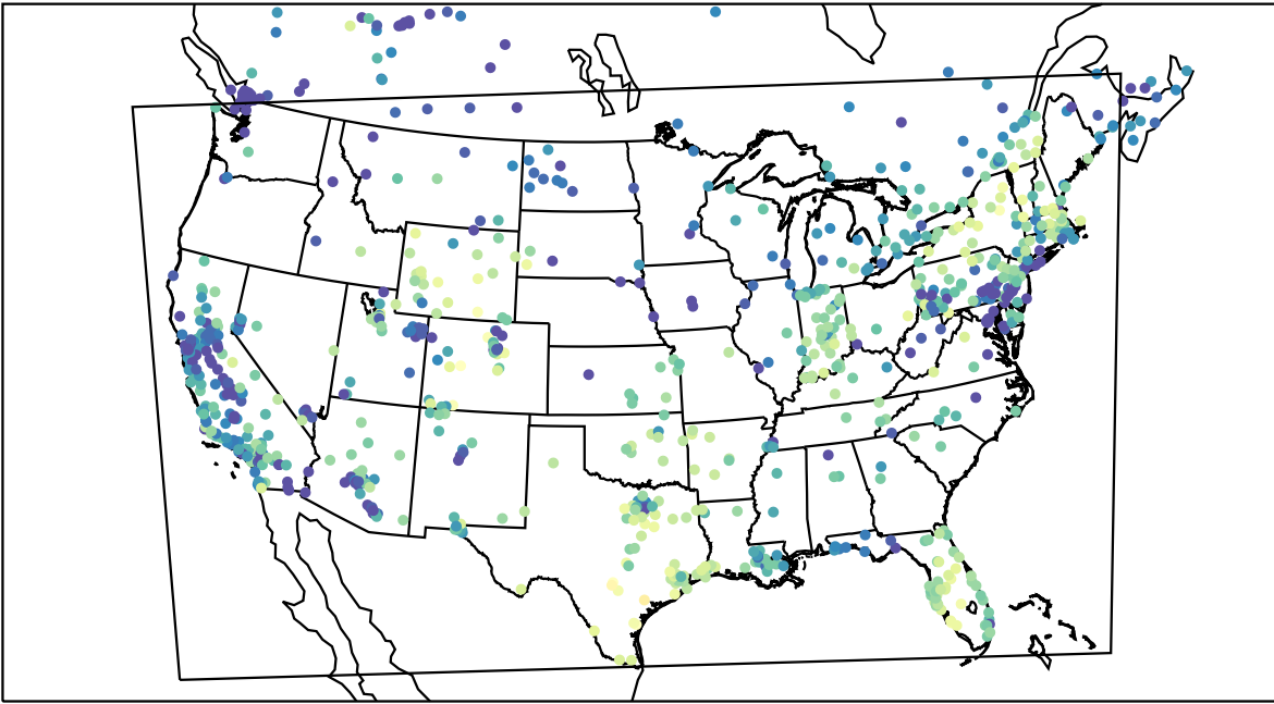
AirNOW (2019-12-23_19:00:00)
