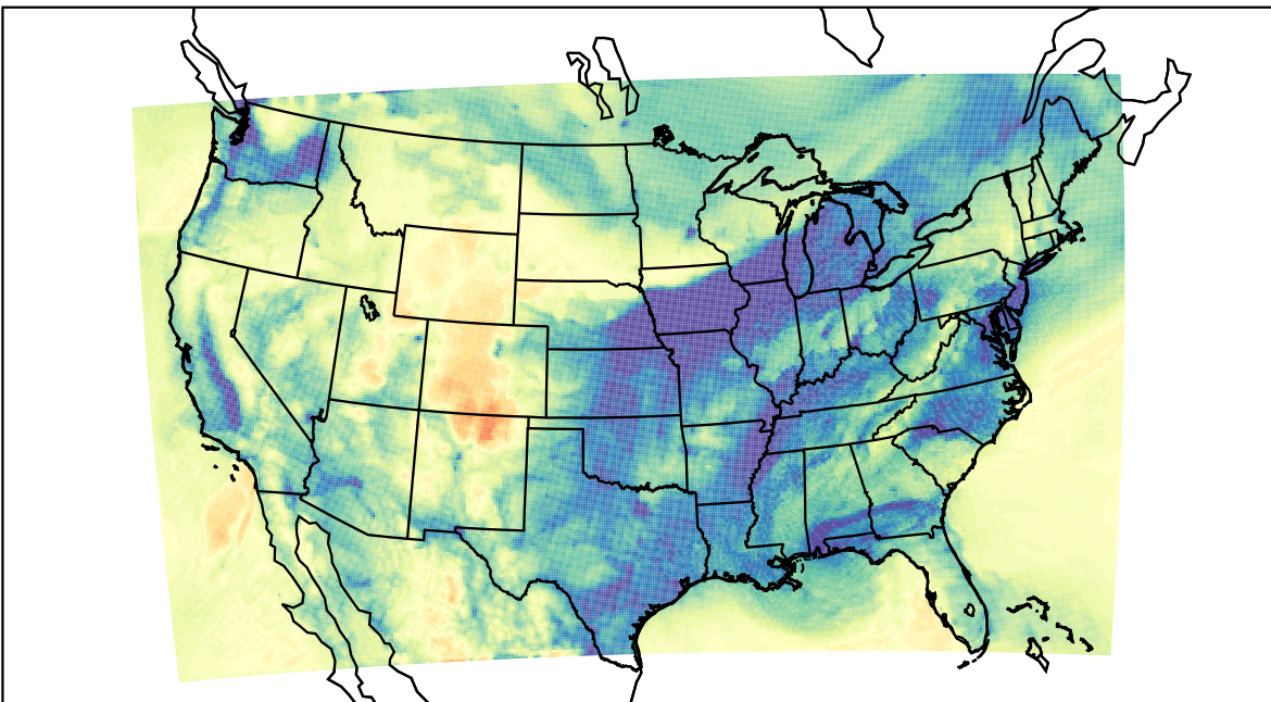
WRF (2019-12-23_15:00:00)
