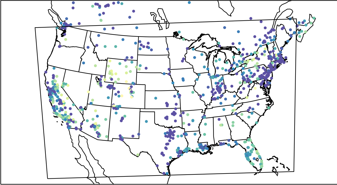
AirNOW (2019-12-23_03:00:00)
