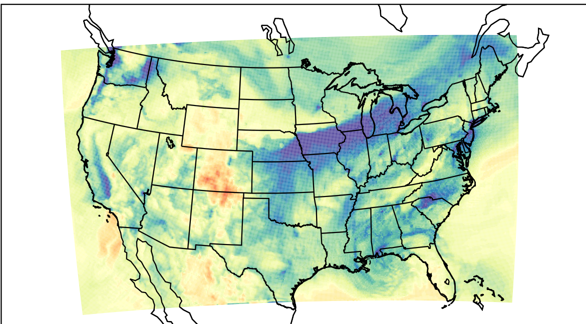
WRF (2019-12-23_18:00:00)
