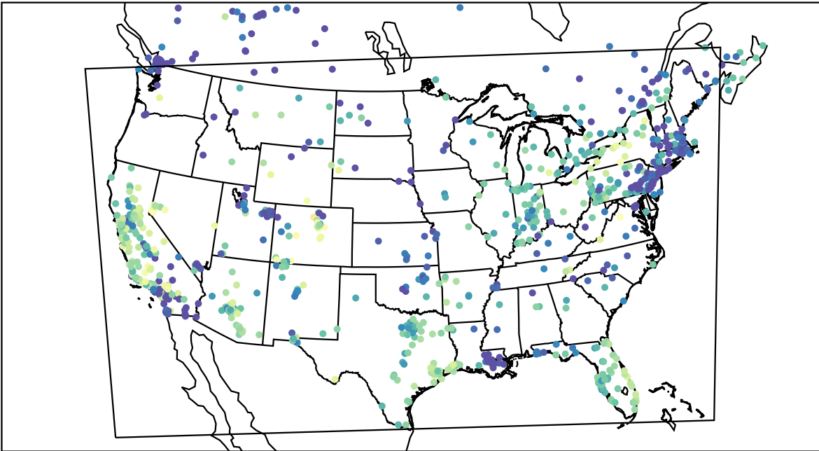
AirNOW (2019-12-22_18:00:00)
