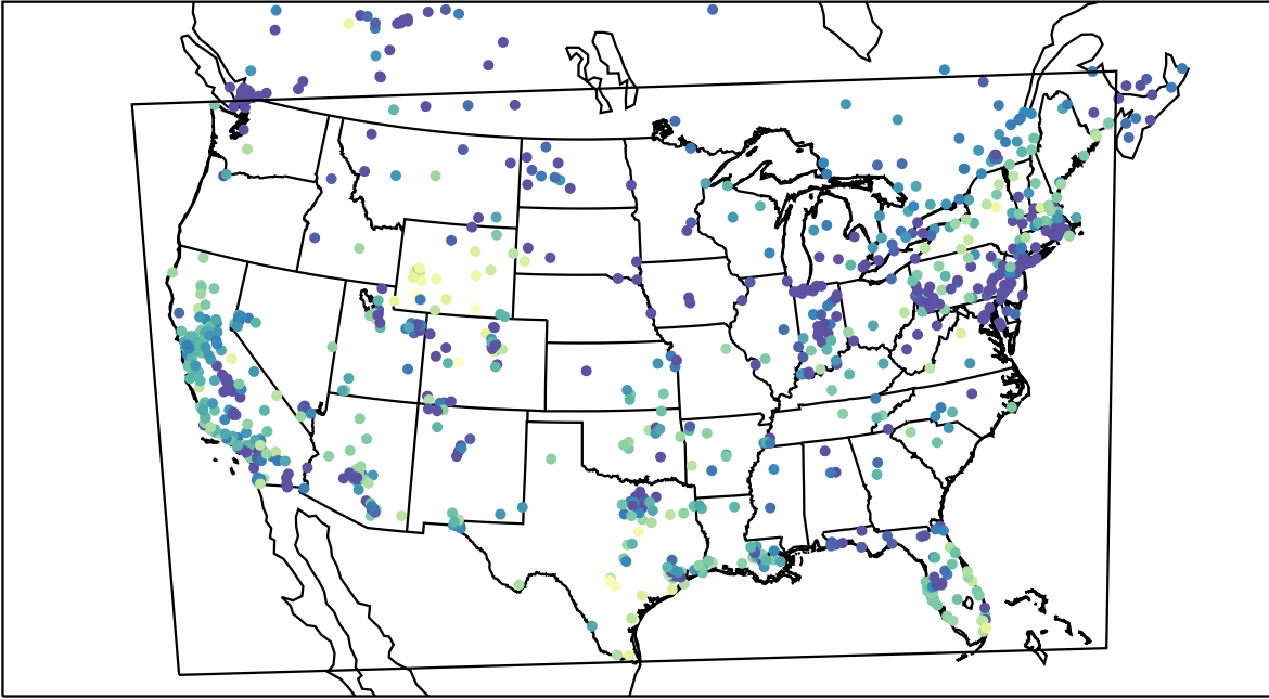
AirNOW (2019-12-23_23:00:00)
