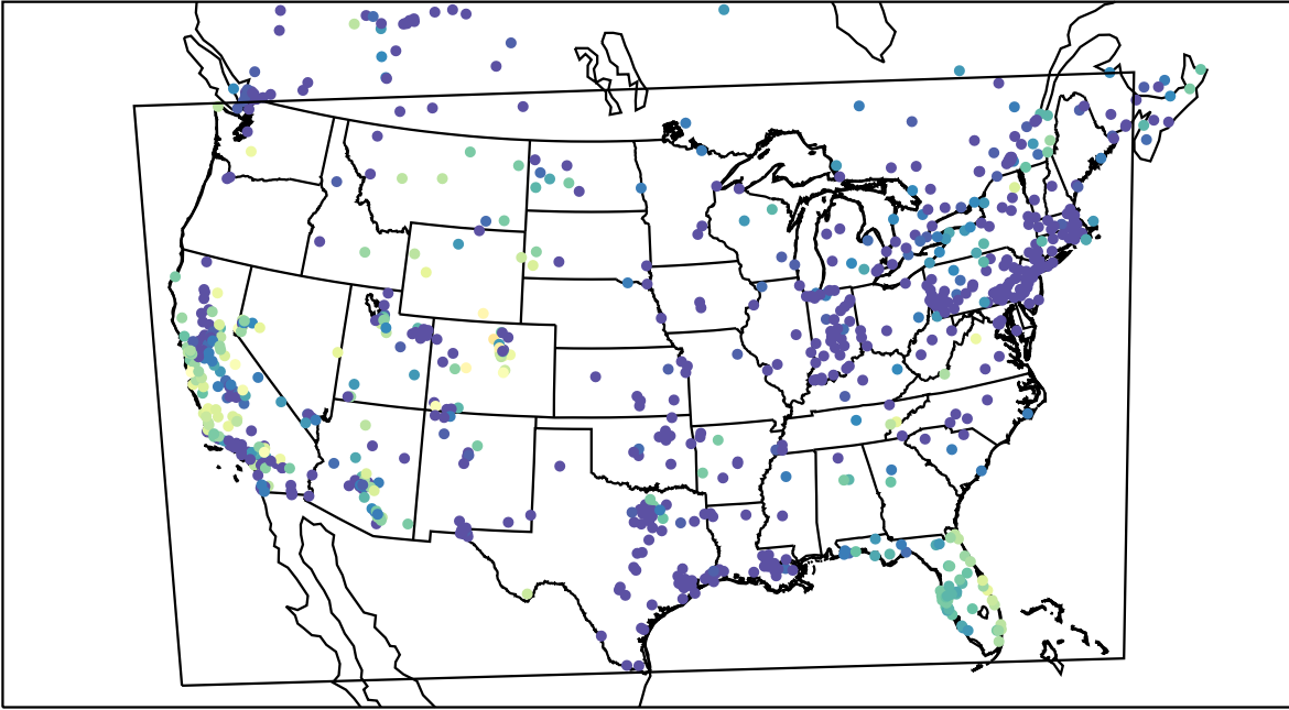
AirNOW (2019-12-22_14:00:00)
