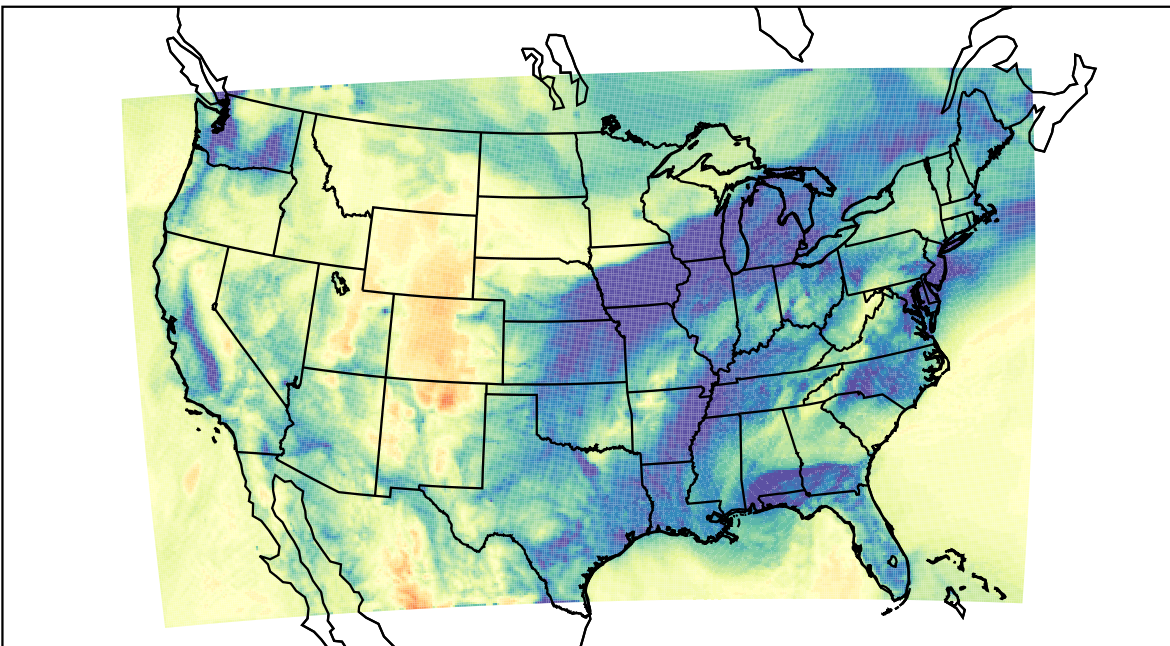
WRF (2019-12-23_12:00:00)
