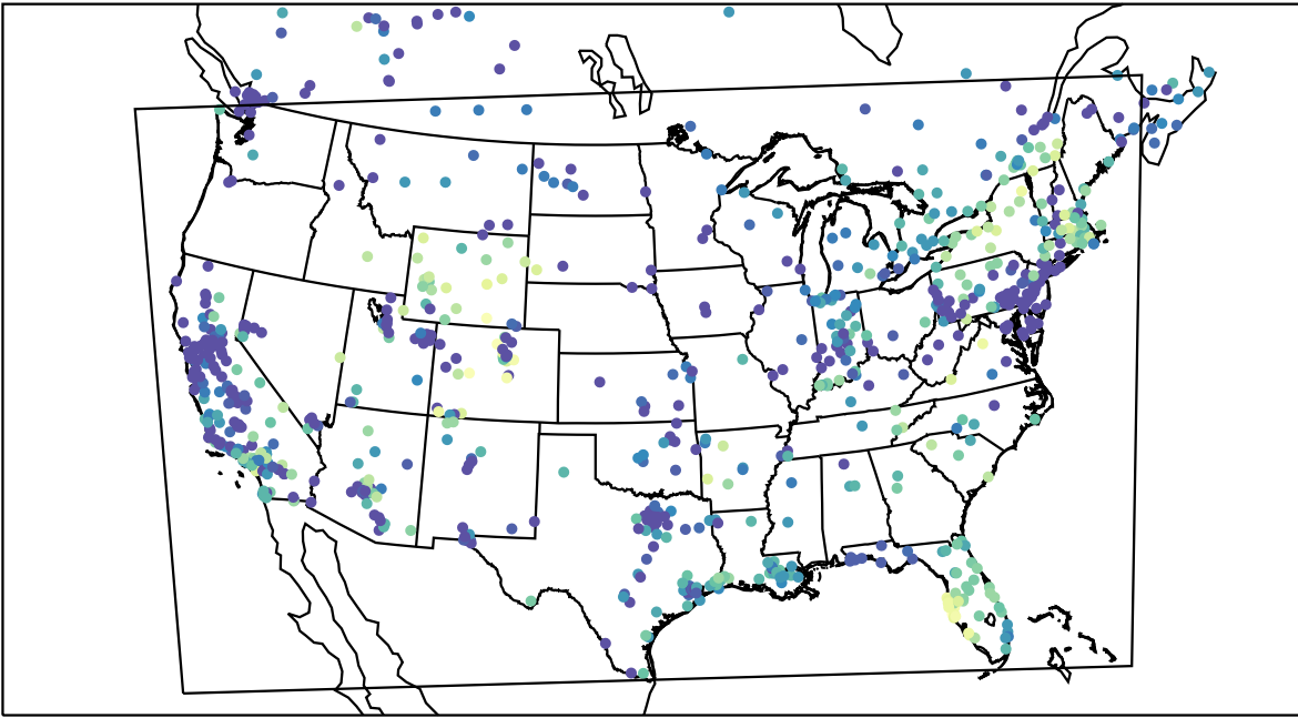
AirNOW (2019-12-23_16:00:00)
