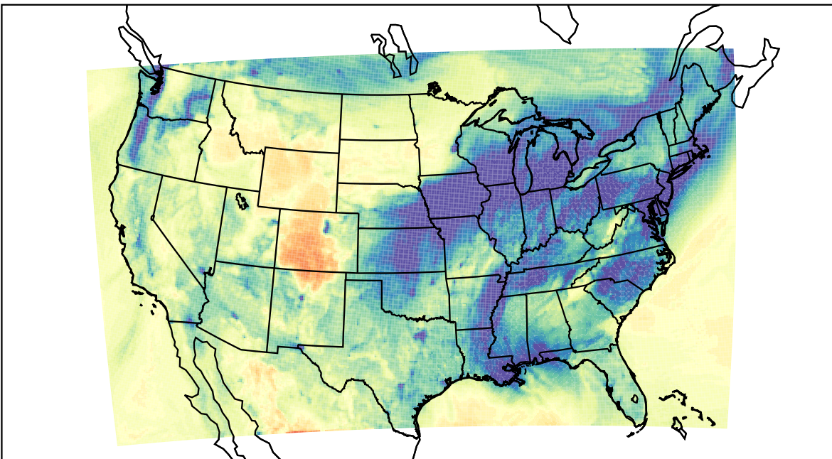
WRF (2019-12-23_00:00:00)
