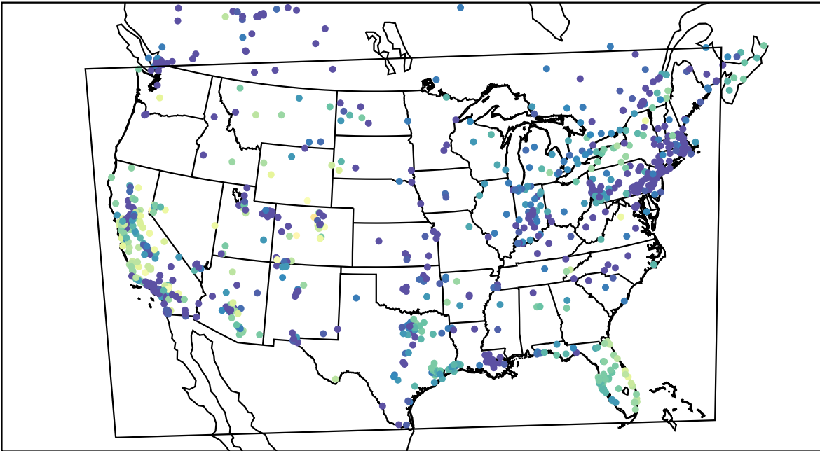
AirNOW (2019-12-22_16:00:00)
