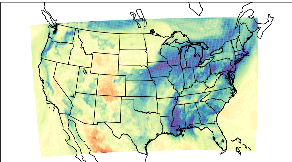
WRF (2019-12-22_20:00:00)
