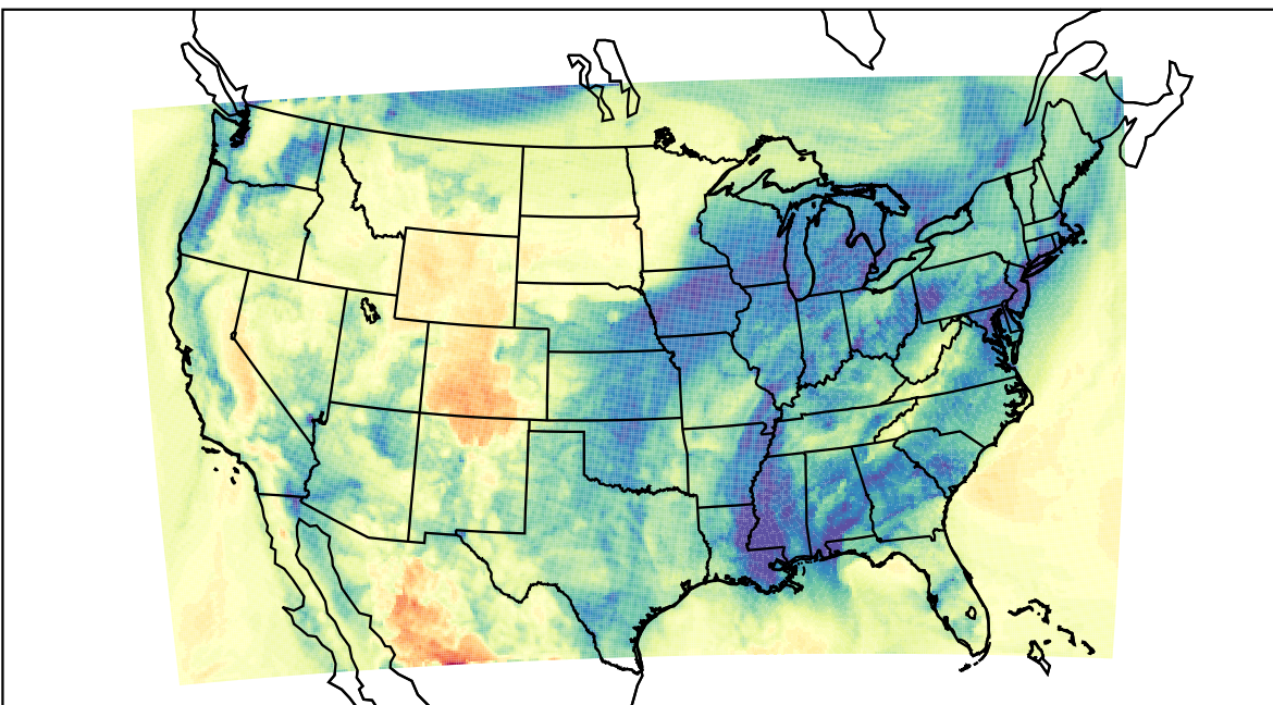
WRF (2019-12-22_18:00:00)
