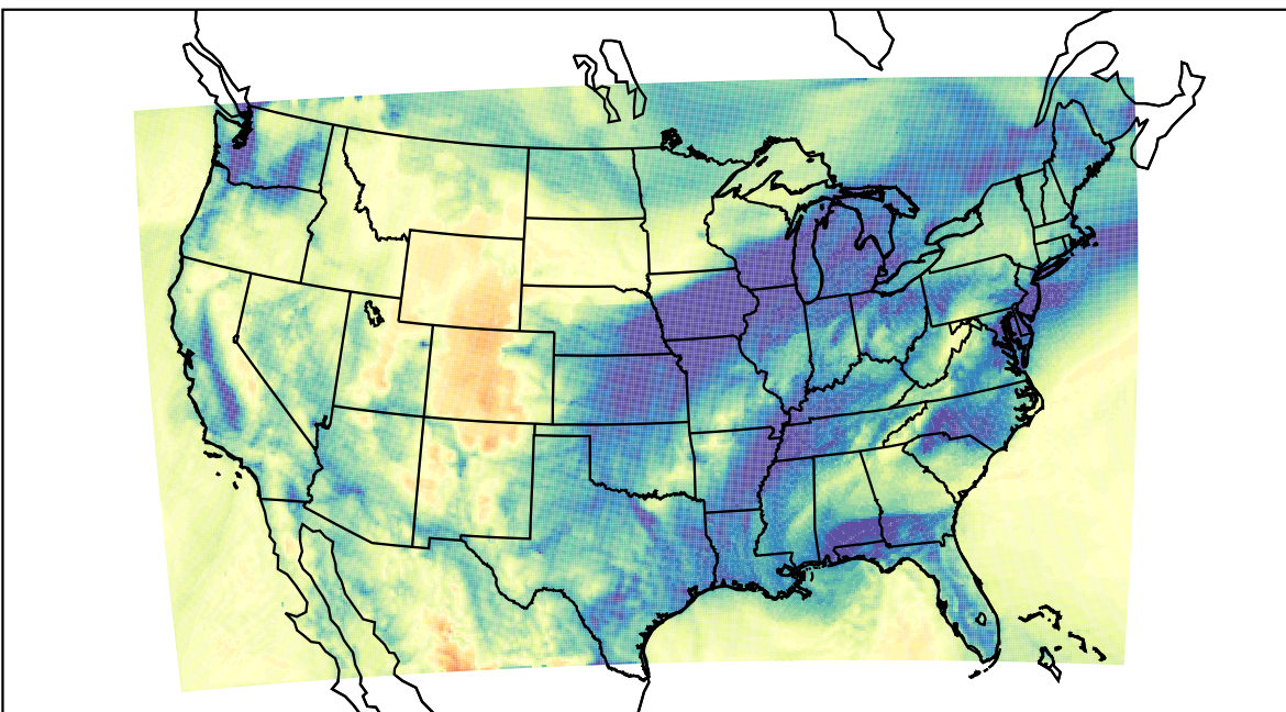
WRF (2019-12-23_10:00:00)
