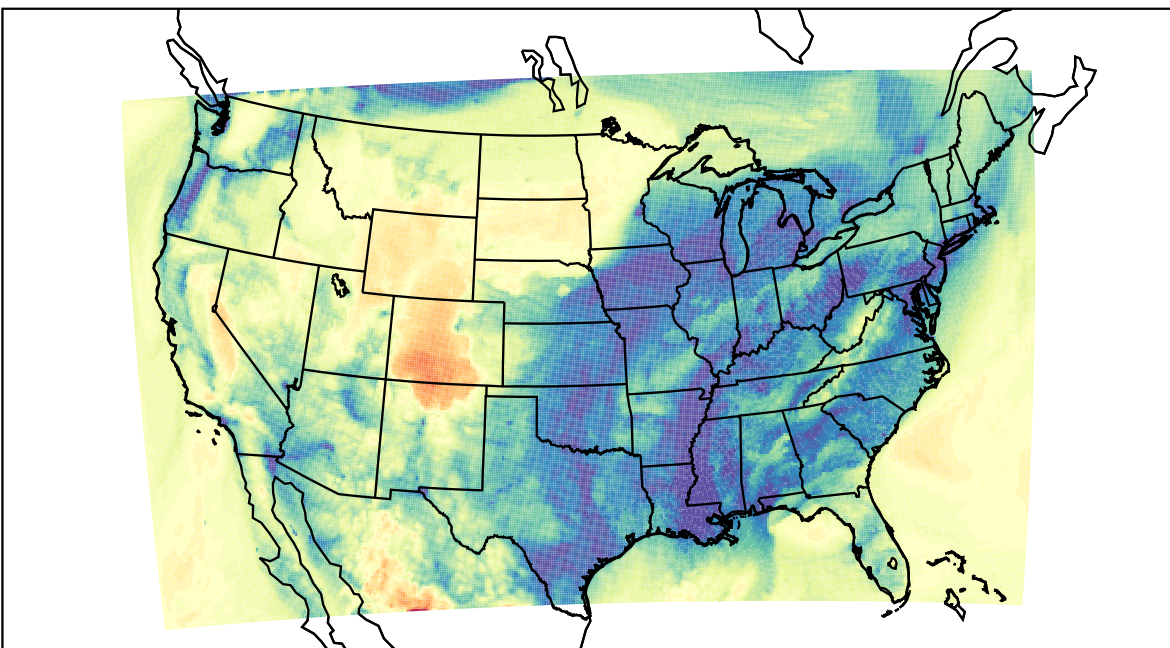
WRF (2019-12-22_16:00:00)
