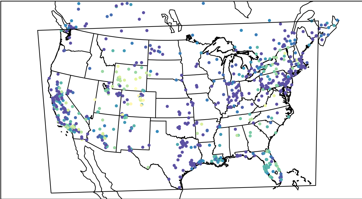
AirNOW (2019-12-23_10:00:00)
