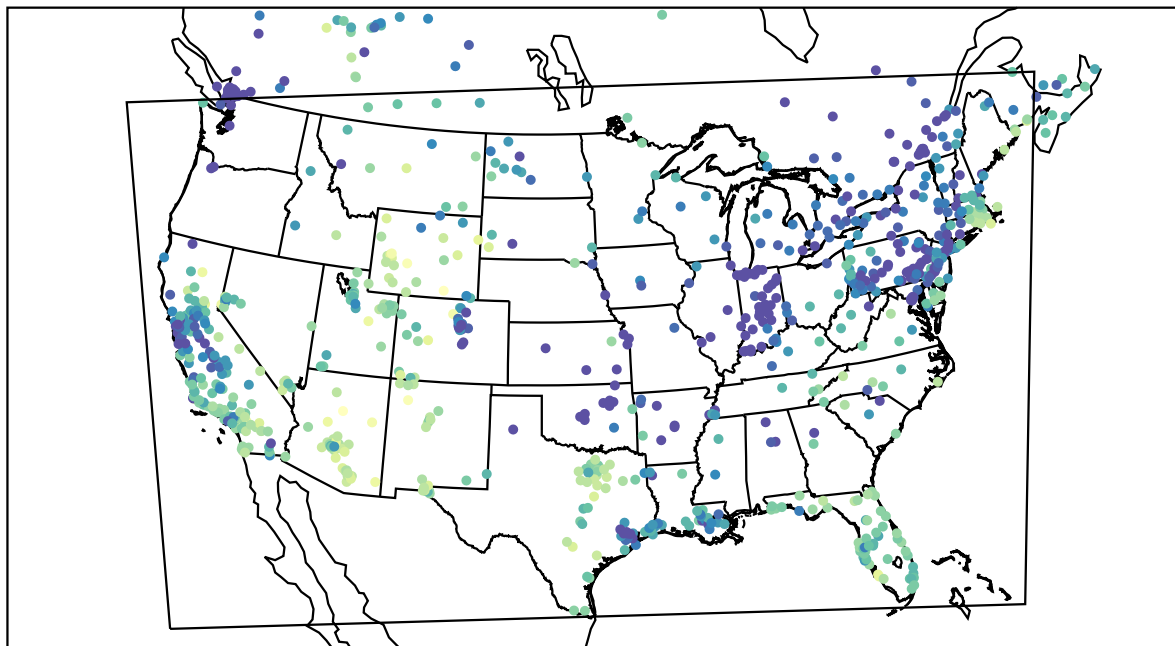
AirNOW (2019-12-27_20:00:00)
