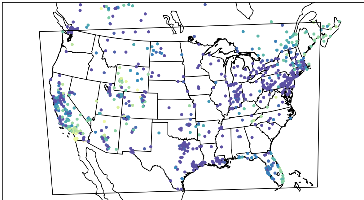
AirNOW (2019-12-26_14:00:00)
