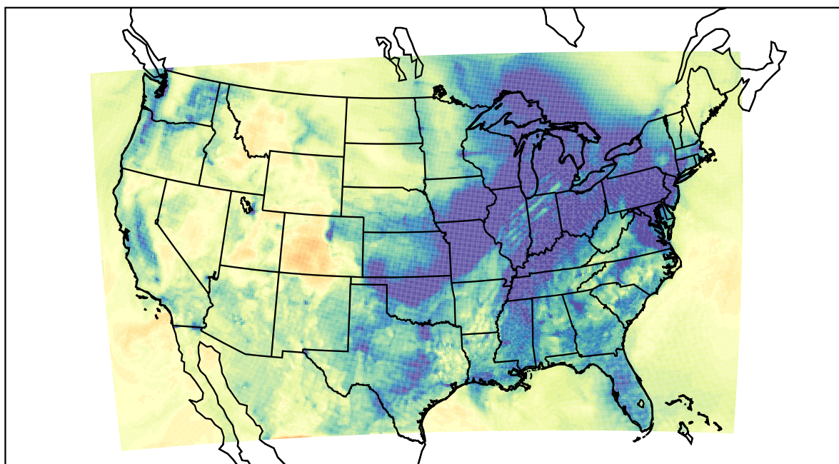
WRF (2019-12-27_01:00:00)
