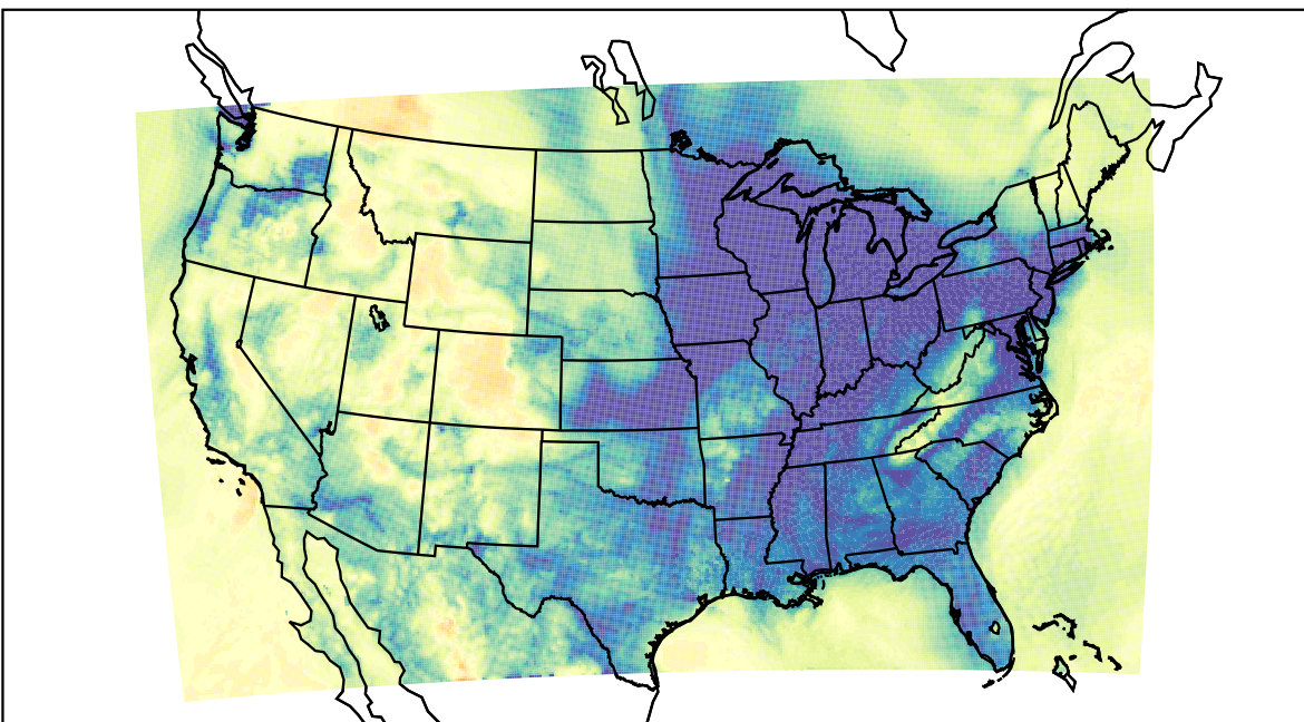
WRF (2019-12-26_12:00:00)
