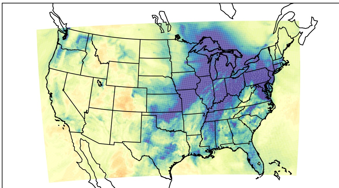
WRF (2019-12-26_23:00:00)
