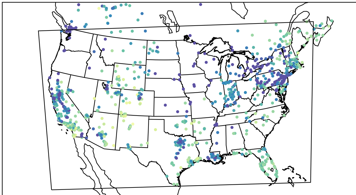
AirNOW (2019-12-26_18:00:00)
