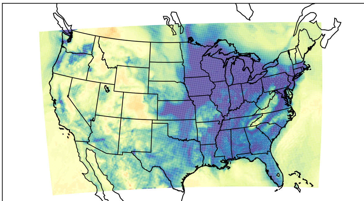
WRF (2019-12-26_10:00:00)
