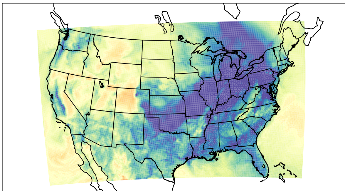
WRF (2019-12-27_08:00:00)
