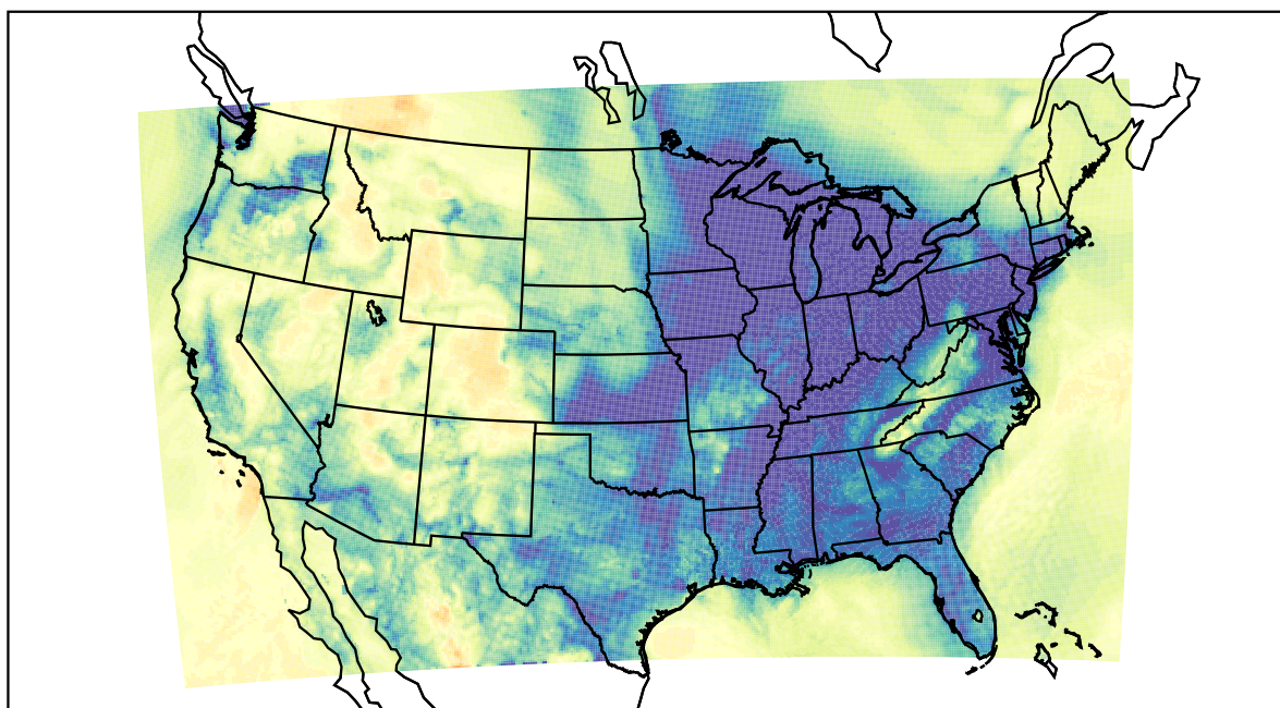
WRF (2019-12-26_13:00:00)
