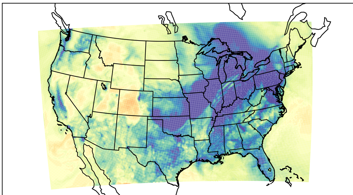
WRF (2019-12-27_03:00:00)
