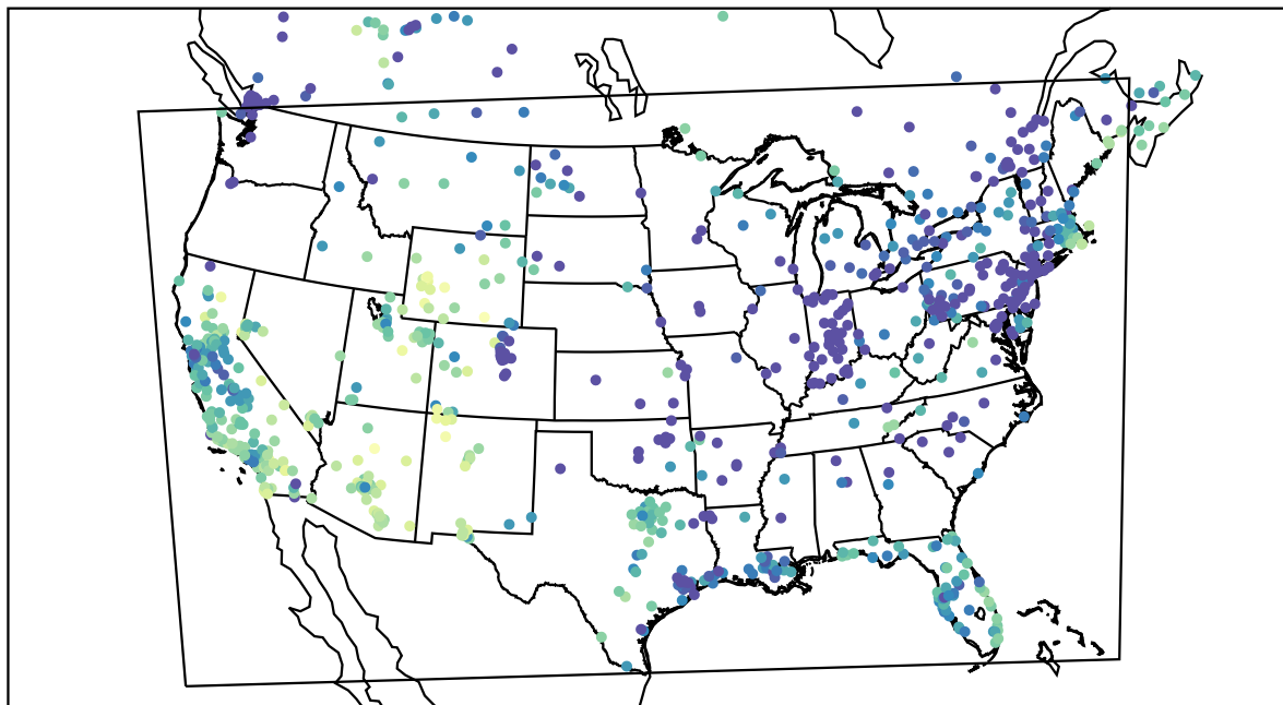
AirNOW (2019-12-27_23:00:00)
