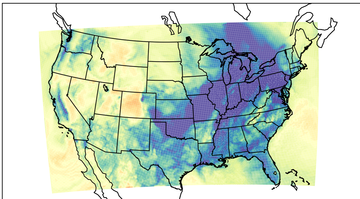
WRF (2019-12-27_06:00:00)
