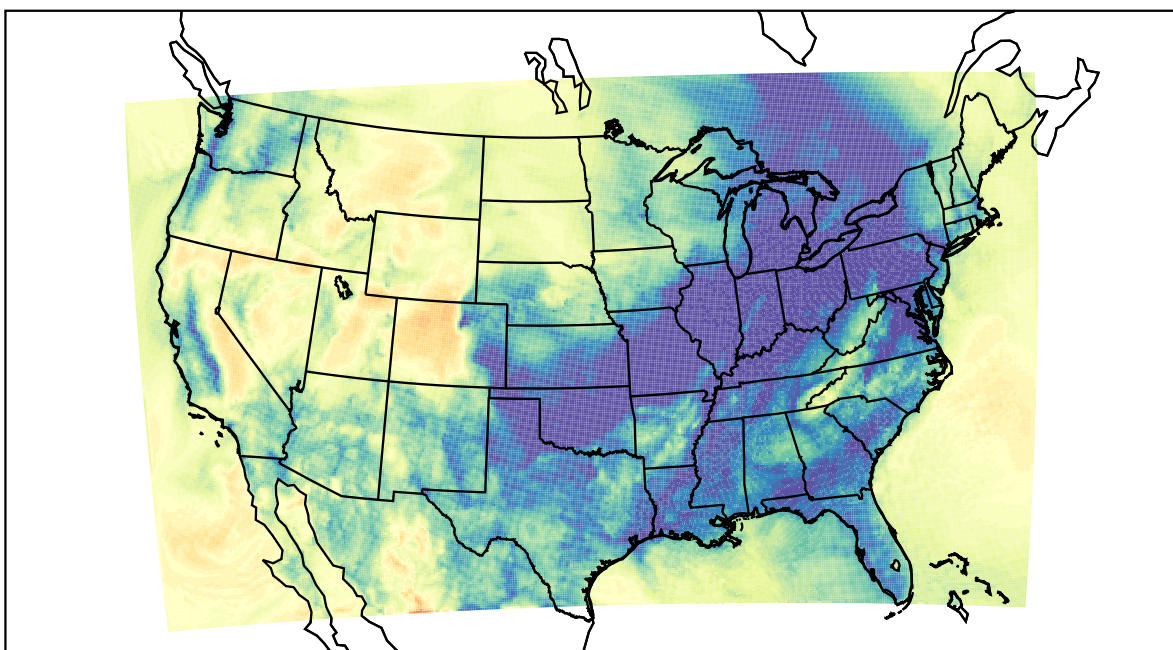
WRF (2019-12-27_09:00:00)
