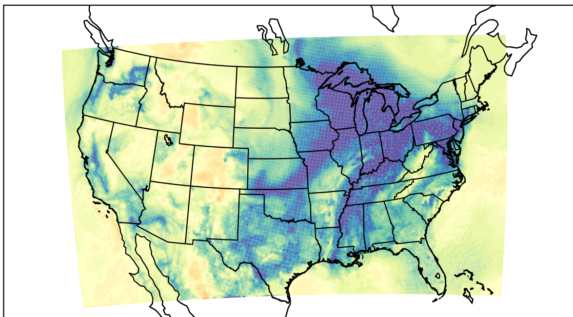
WRF (2019-12-26_17:00:00)
