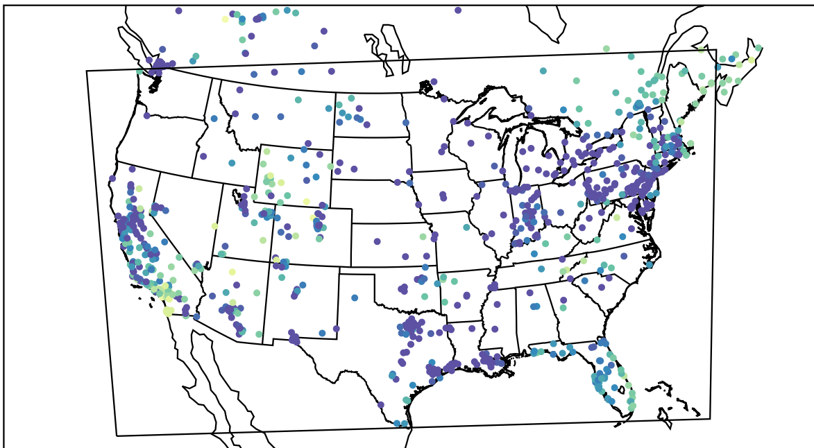
AirNOW (2019-12-26_15:00:00)
