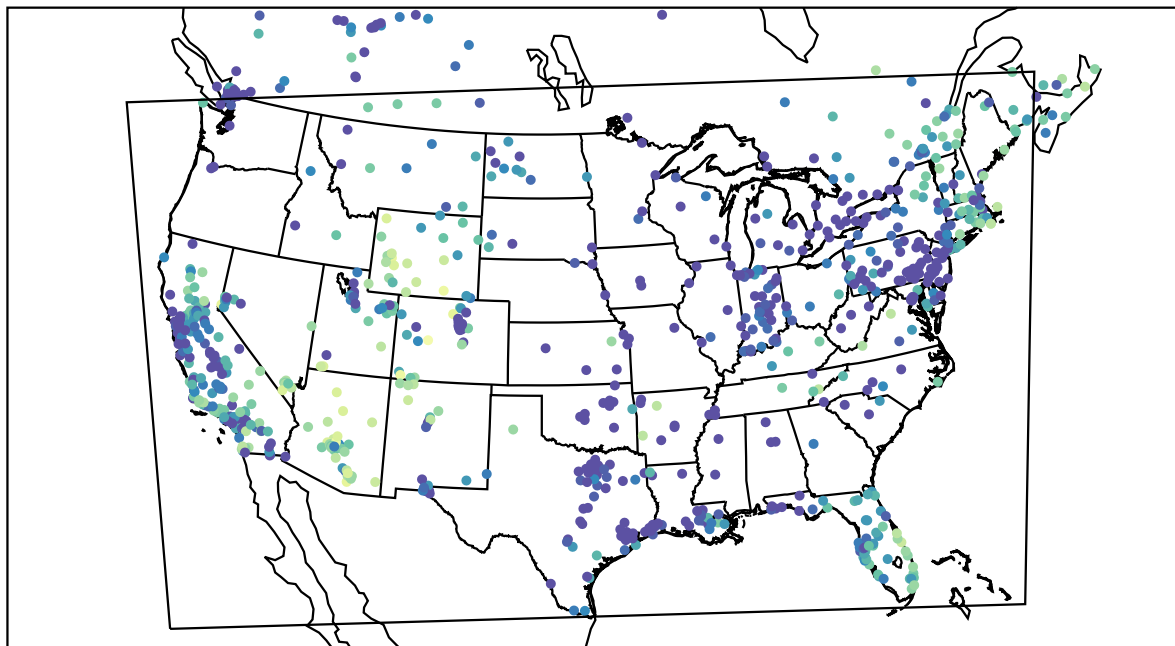
AirNOW (2019-12-27_01:00:00)
