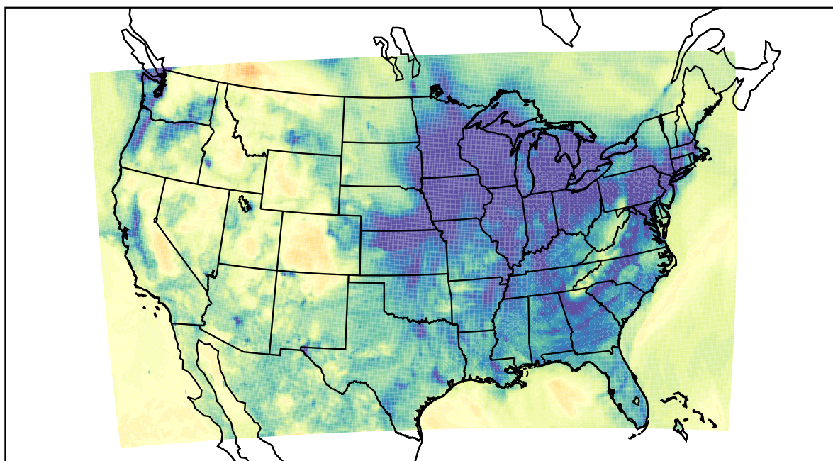
WRF (2019-12-26_04:00:00)
