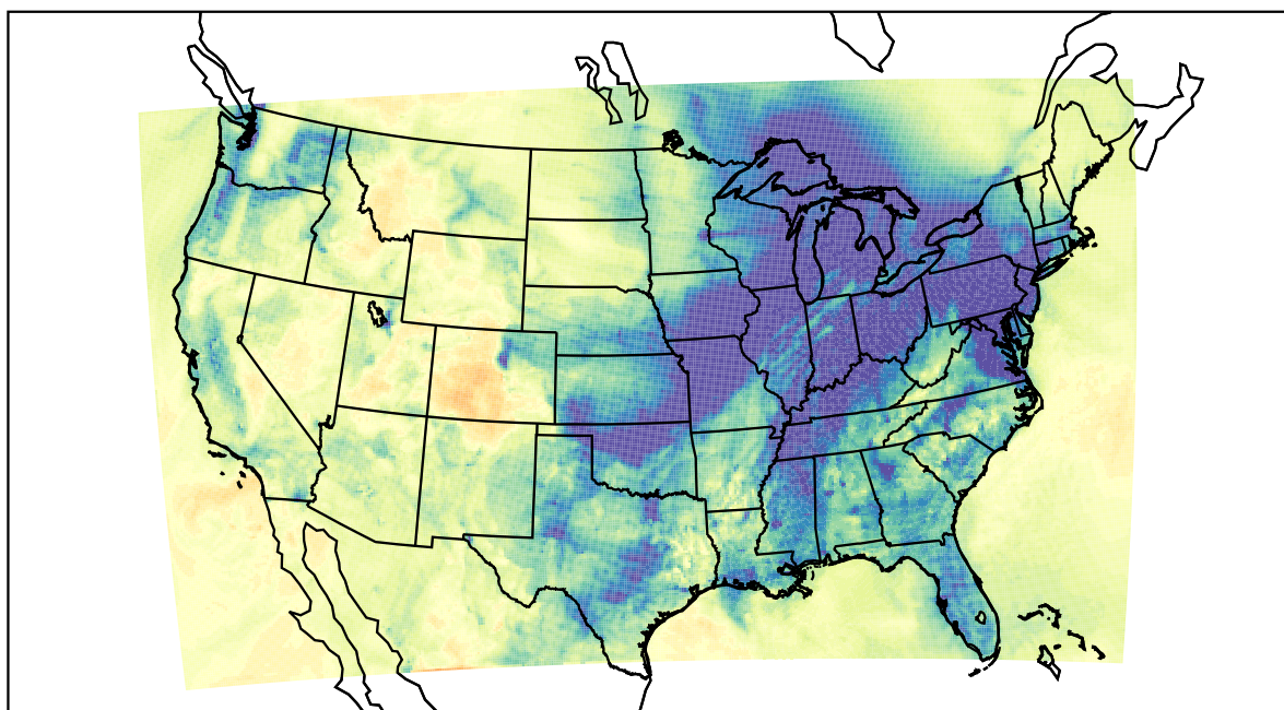
WRF (2019-12-27_00:00:00)
