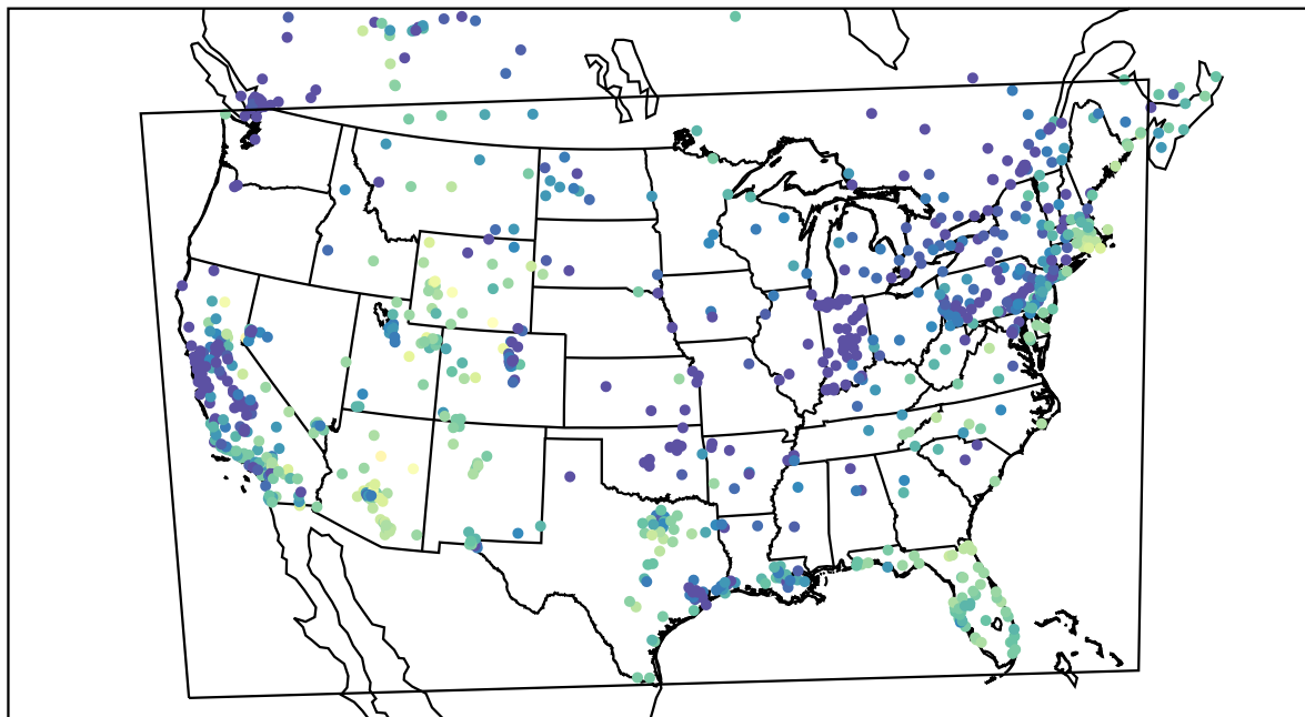
AirNOW (2019-12-27_18:00:00)
