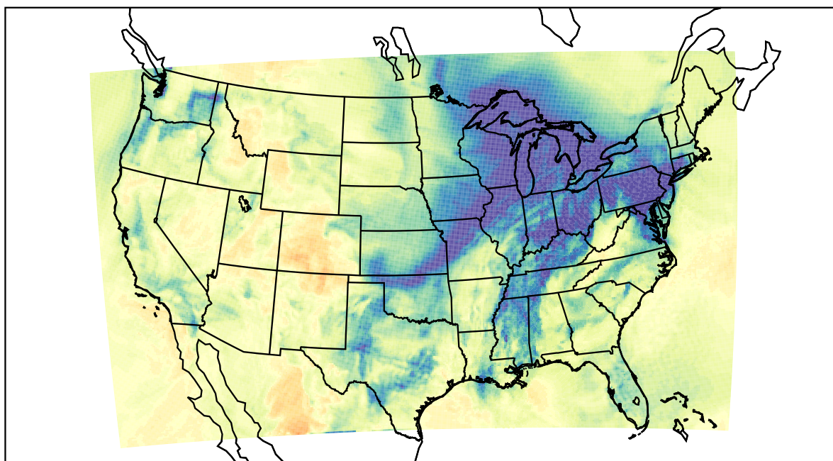
WRF (2019-12-26_20:00:00)
