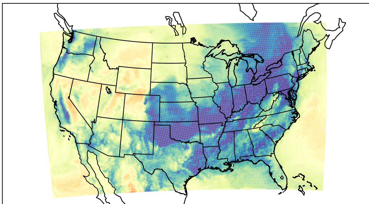
WRF (2019-12-27_16:00:00)
