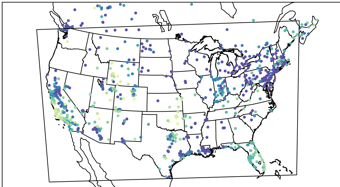
AirNOW (2019-12-26_03:00:00)
