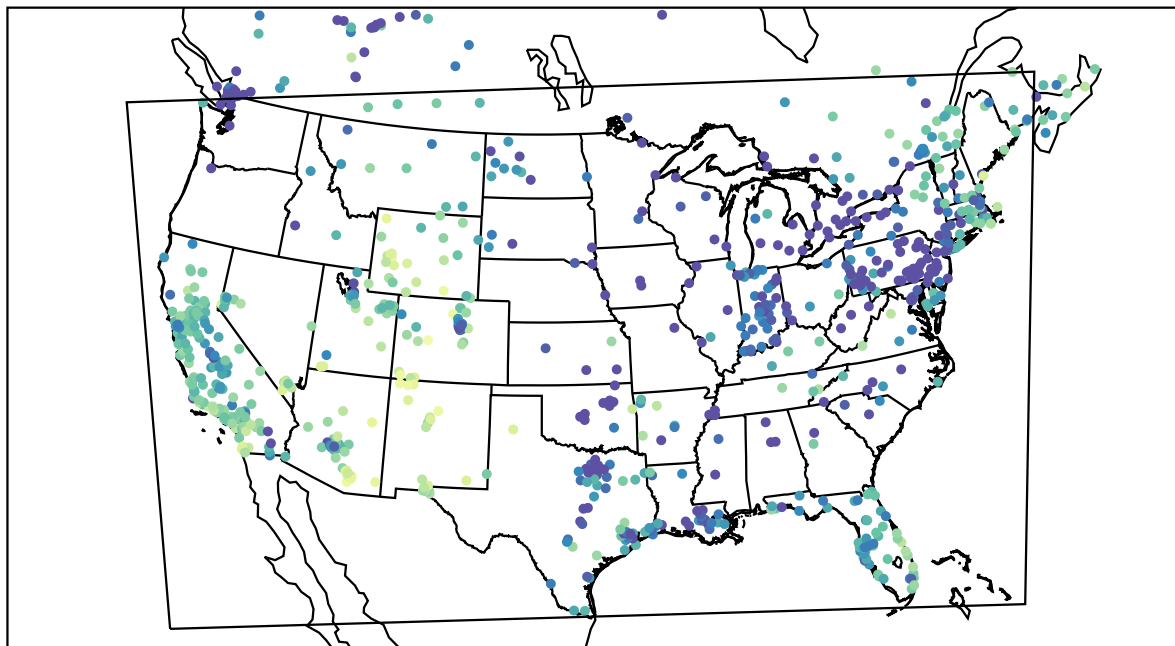
AirNOW (2019-12-26_23:00:00)
