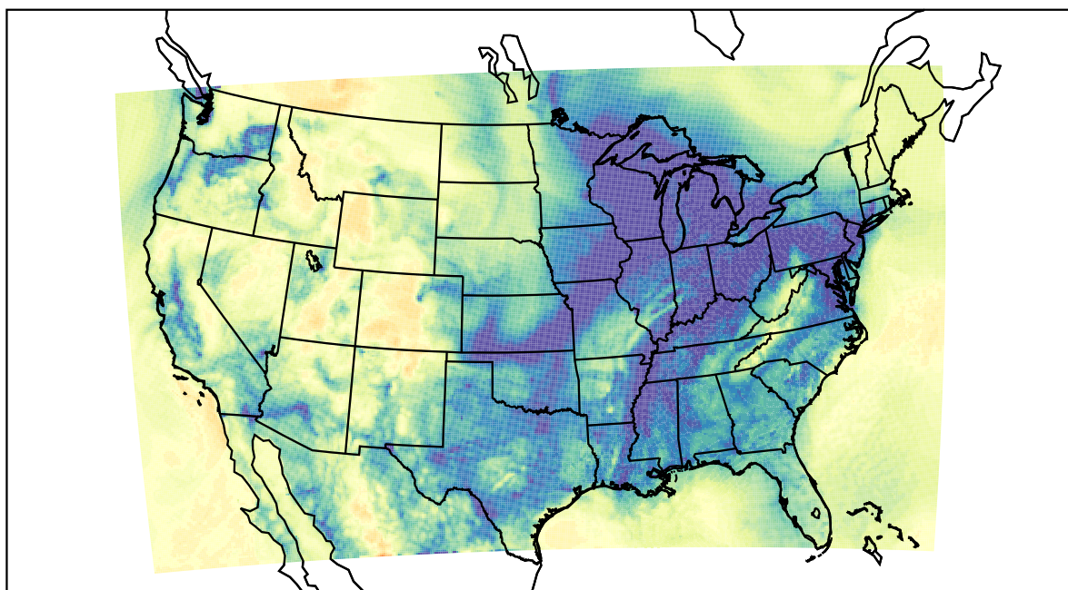
WRF (2019-12-26_16:00:00)
