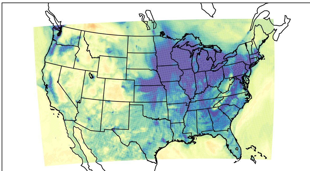
WRF (2019-12-26_03:00:00)
