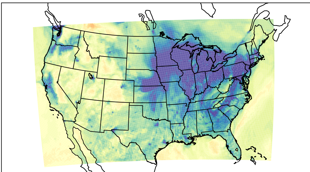
WRF (2019-12-26_01:00:00)
