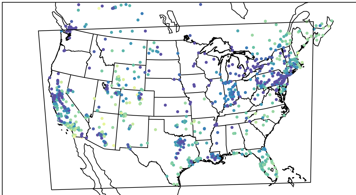
AirNOW (2019-12-26_17:00:00)
