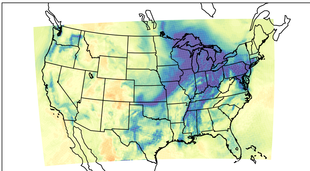
WRF (2019-12-26_19:00:00)
