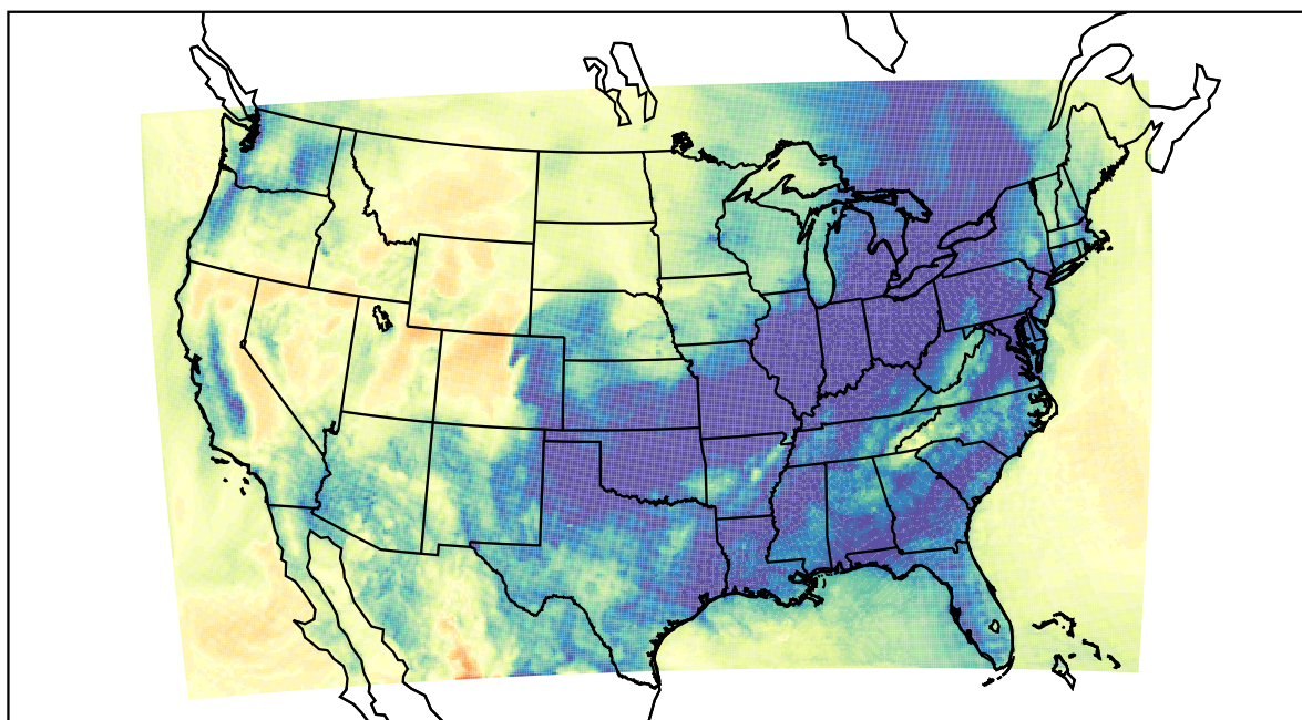
WRF (2019-12-27_13:00:00)
