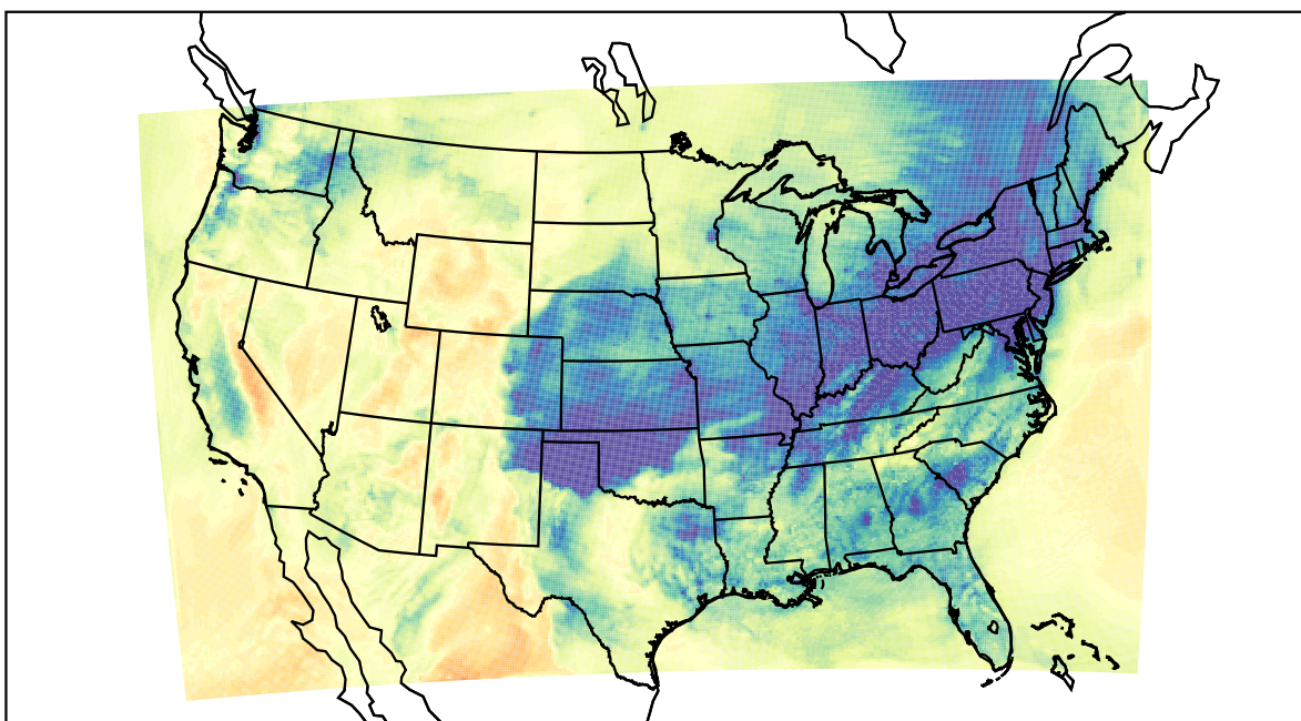
WRF (2019-12-27_22:00:00)
