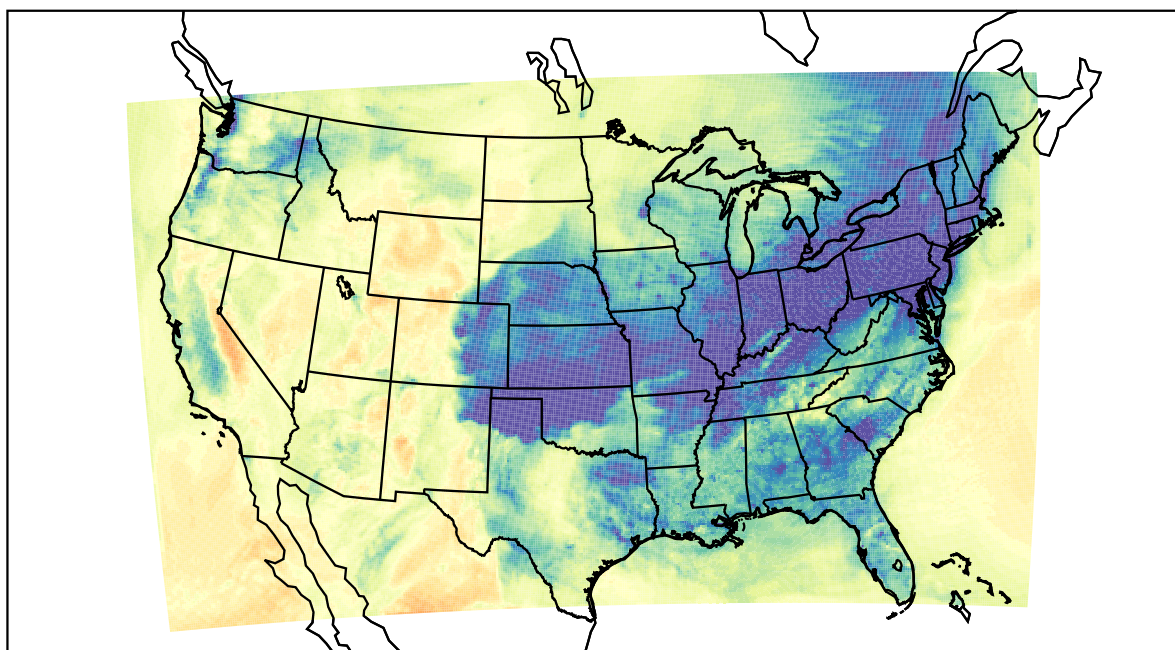
WRF (2019-12-27_23:00:00)
