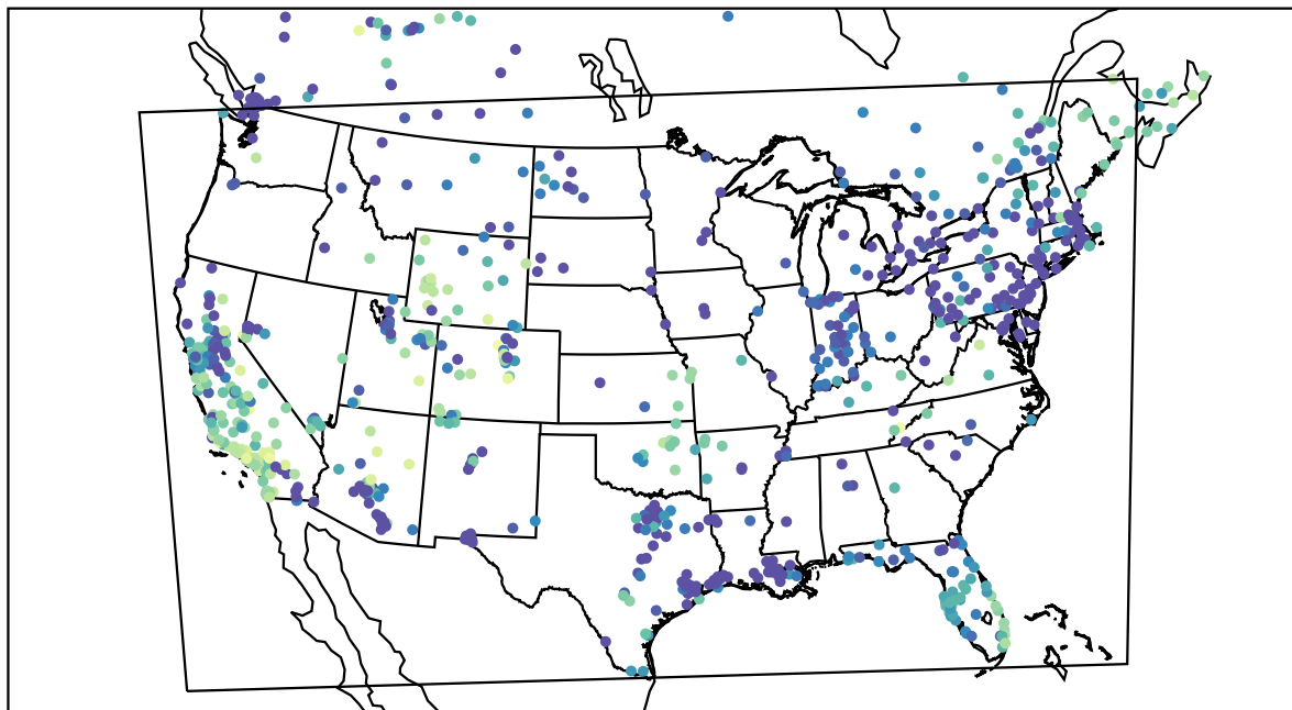
AirNOW (2019-12-26_08:00:00)
