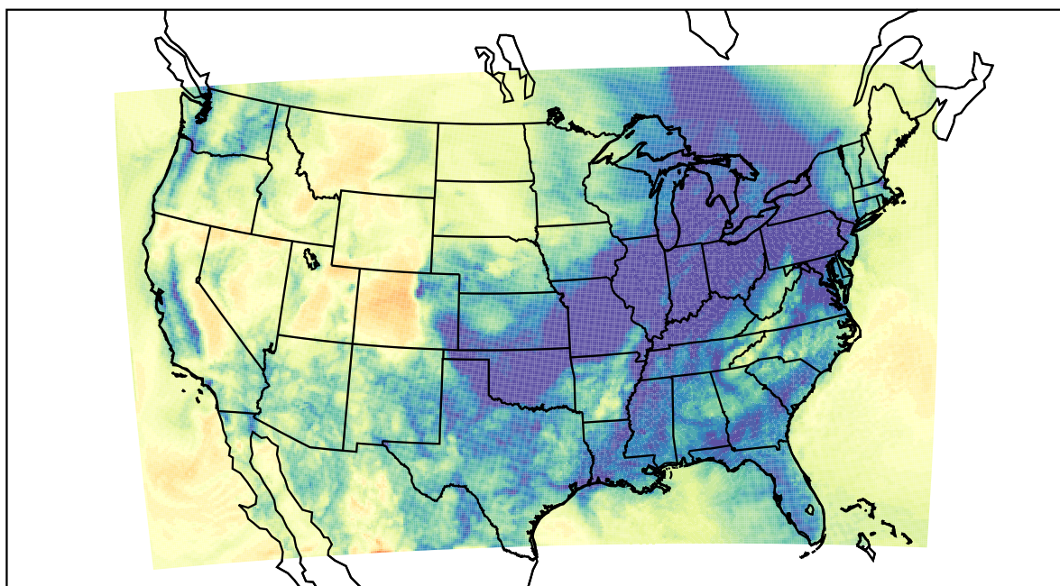
WRF (2019-12-27_07:00:00)
