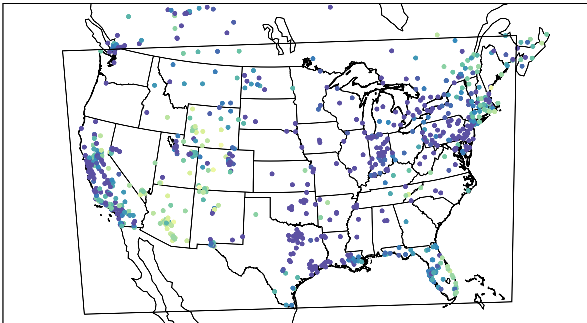
AirNOW (2019-12-27_04:00:00)
