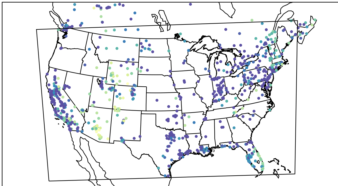
AirNOW (2019-12-27_08:00:00)
