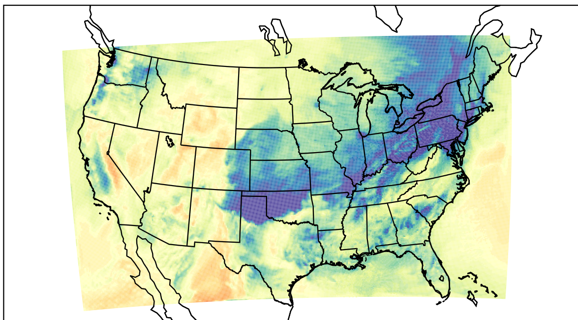
WRF (2019-12-27_20:00:00)
