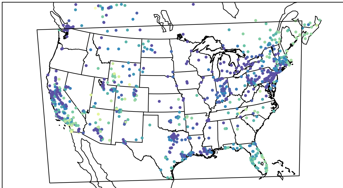
AirNOW (2019-12-26_16:00:00)
