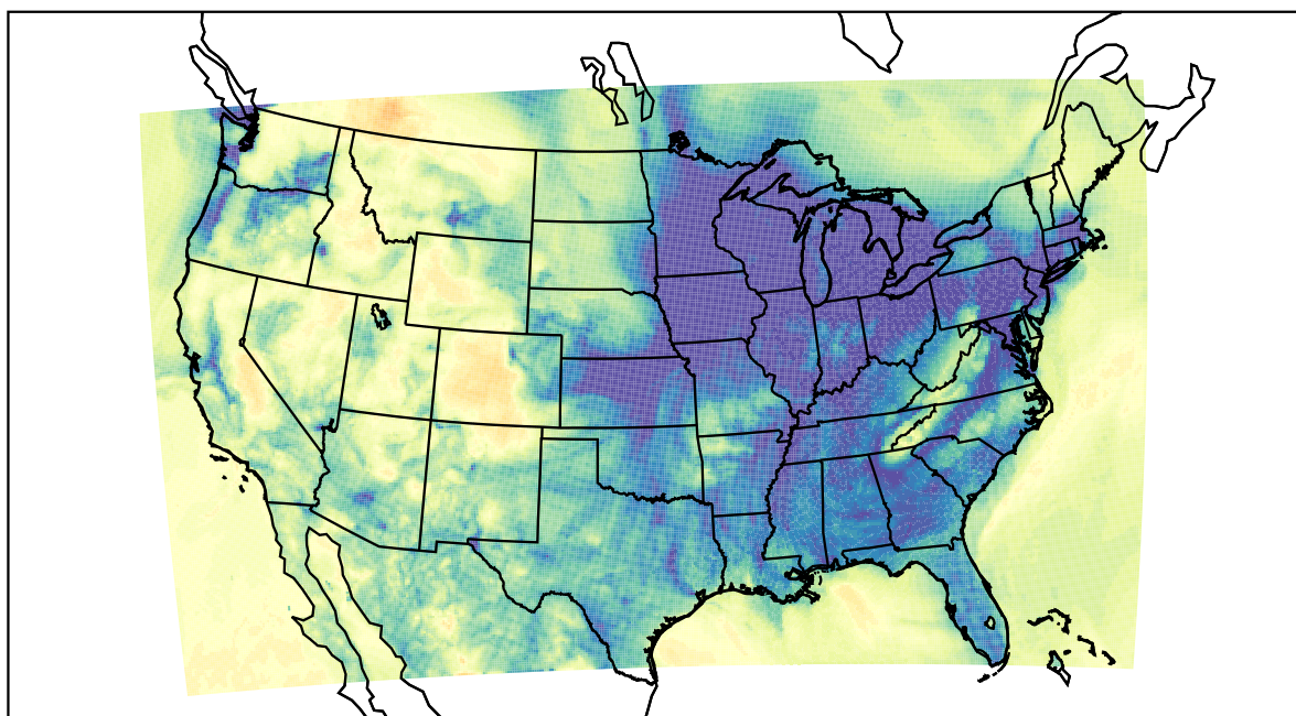
WRF (2019-12-26_07:00:00)
