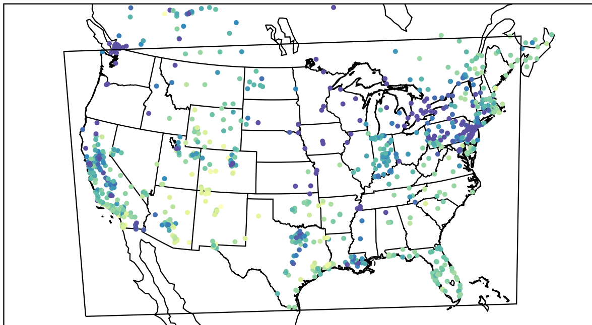
AirNOW (2019-12-26_19:00:00)
