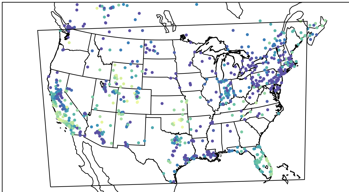
AirNOW (2019-12-26_04:00:00)
