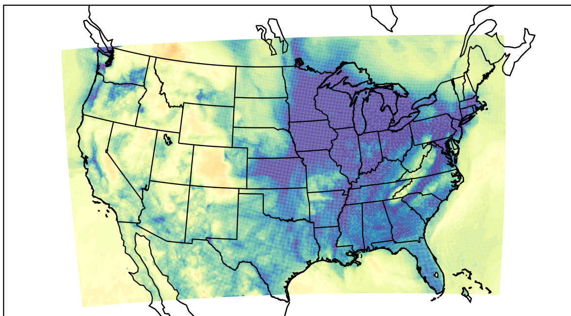
WRF (2019-12-26_08:00:00)
