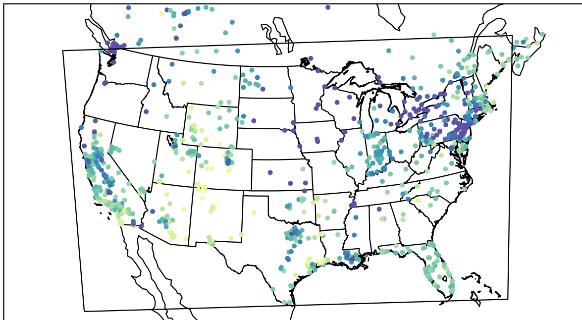
AirNOW (2019-12-26_20:00:00)
