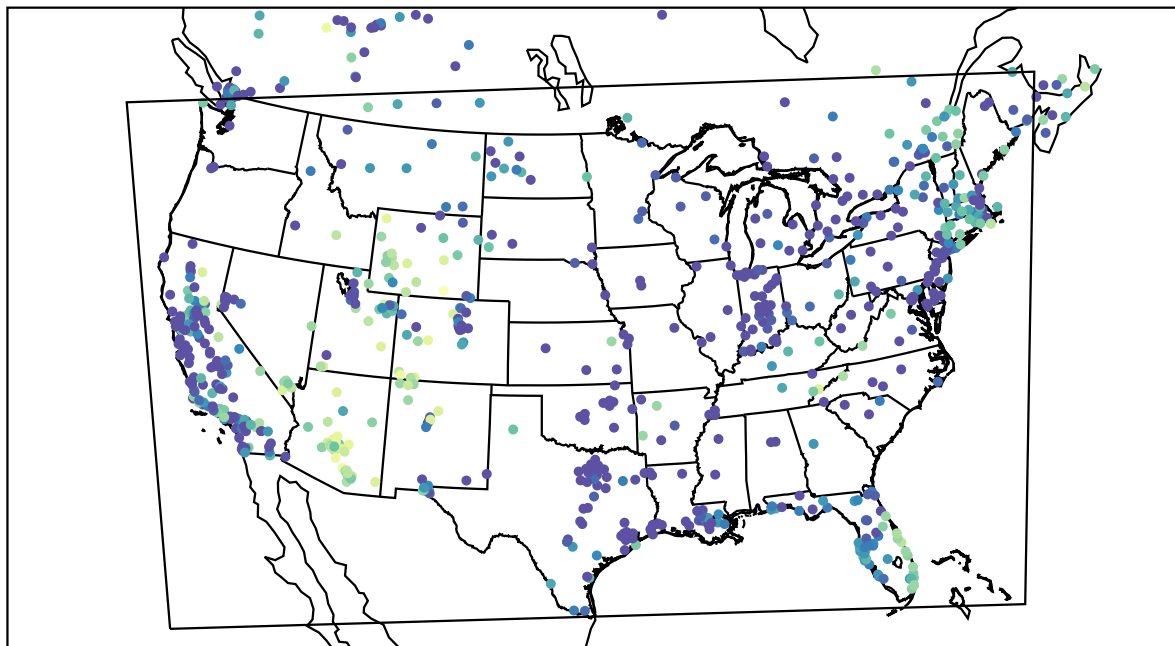
AirNOW (2019-12-27_06:00:00)
