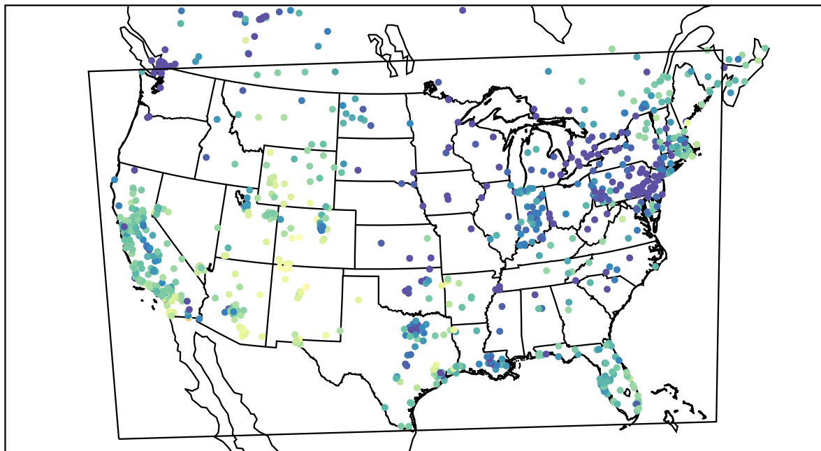
AirNOW (2019-12-26_22:00:00)
