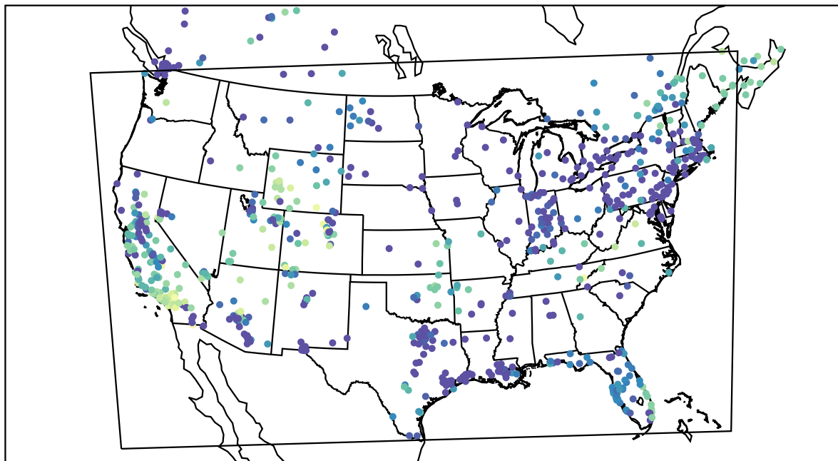
AirNOW (2019-12-26_10:00:00)
