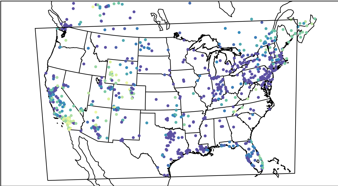
AirNOW (2019-12-26_12:00:00)
