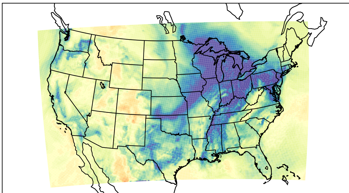
WRF (2019-12-26_18:00:00)
