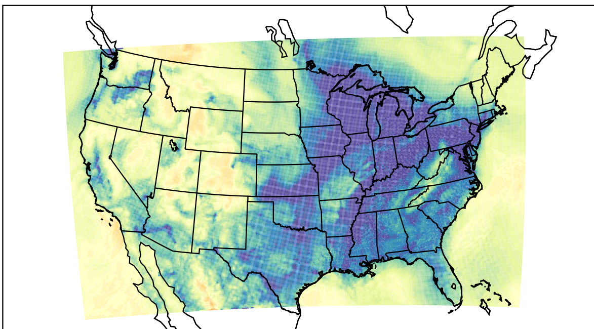
WRF (2019-12-26_15:00:00)
