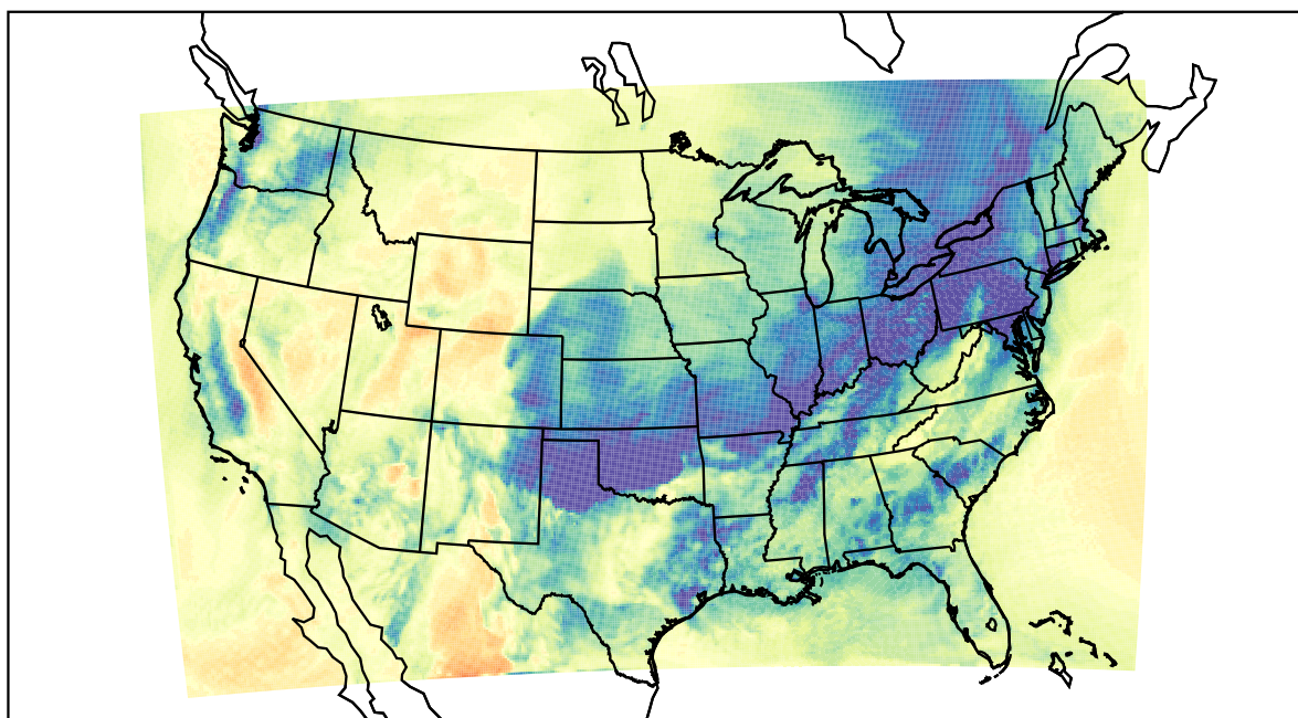
WRF (2019-12-27_18:00:00)
