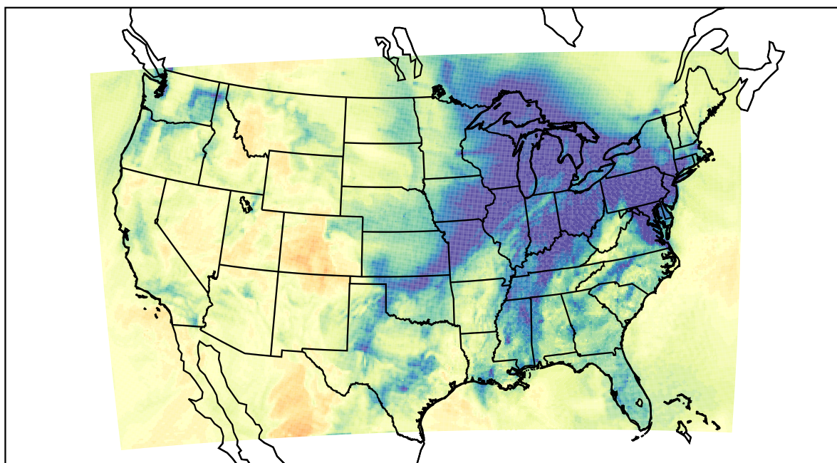
WRF (2019-12-26_22:00:00)
