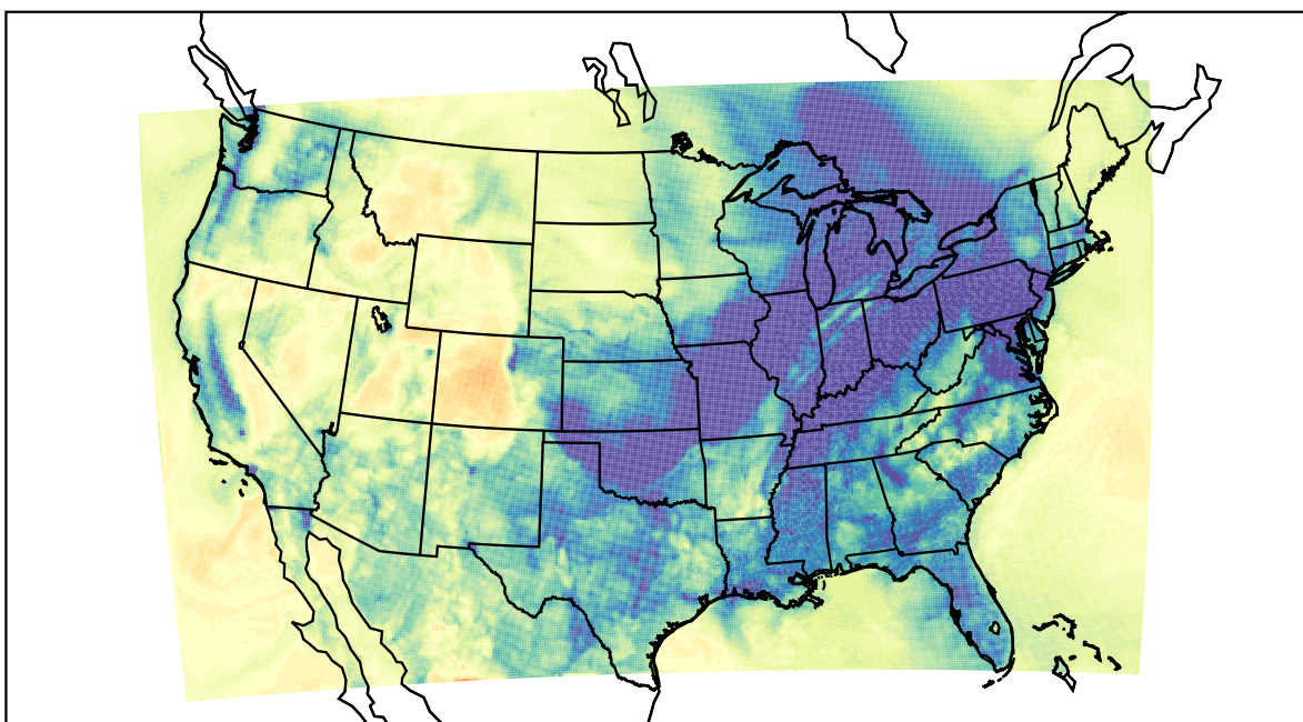
WRF (2019-12-27_04:00:00)
