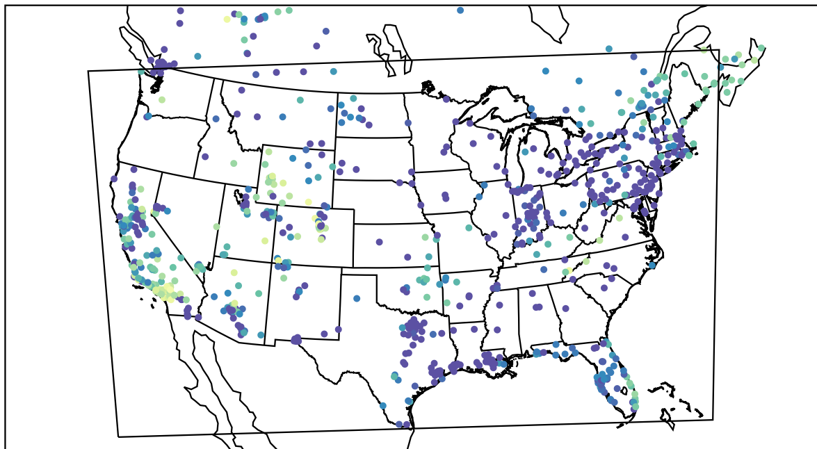
AirNOW (2019-12-26_11:00:00)
