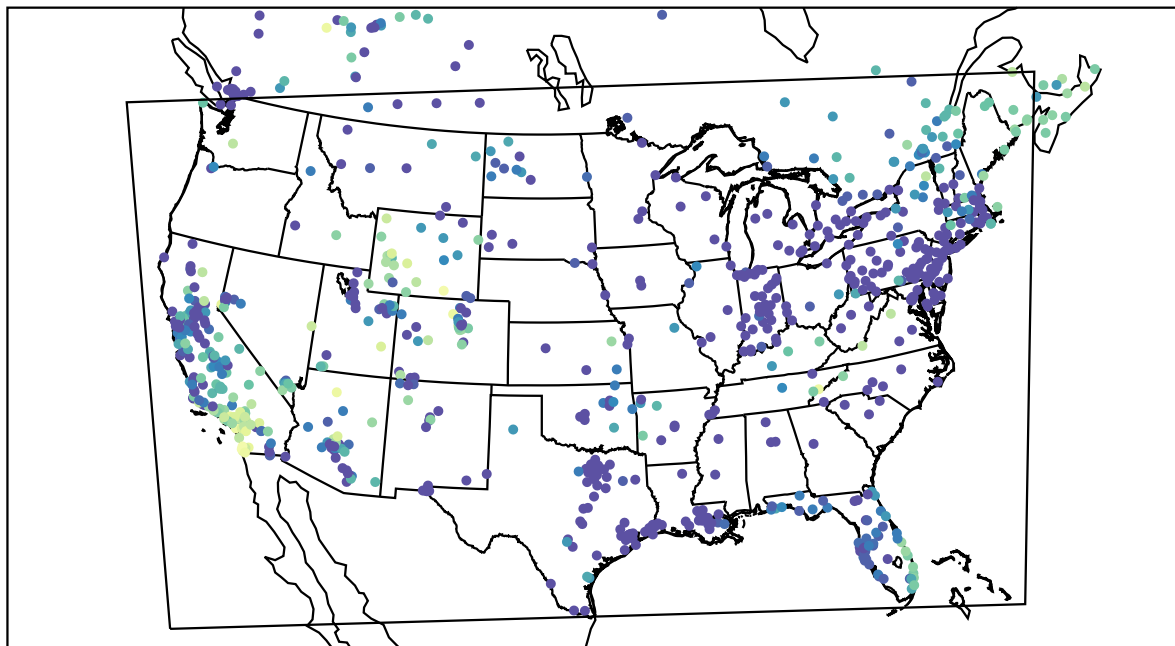
AirNOW (2019-12-26_13:00:00)
