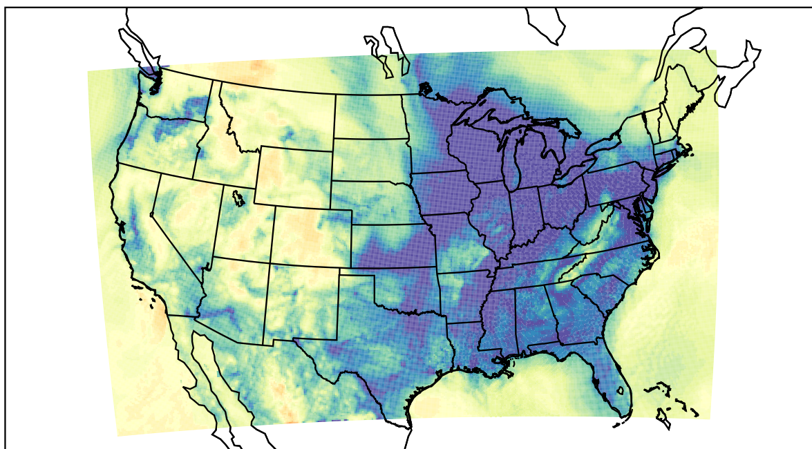
WRF (2019-12-26_14:00:00)
