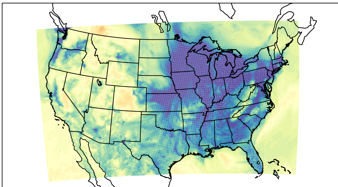
WRF (2019-12-26_06:00:00)
