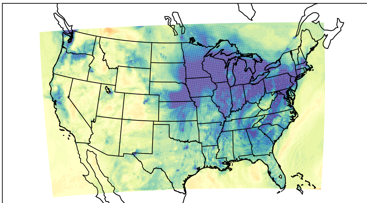
WRF (2019-12-26_00:00:00)
