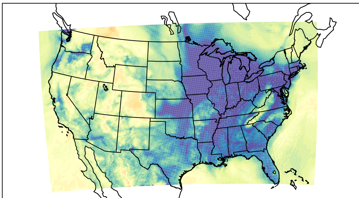
WRF (2019-12-26_11:00:00)
