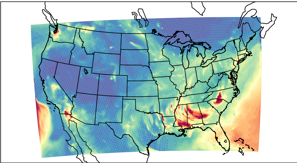
WRF 2020-10-21_08:00:00
