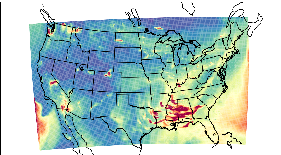
WRF 2020-10-22_04:00:00
