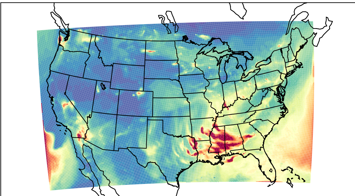
WRF 2020-10-22_06:00:00
