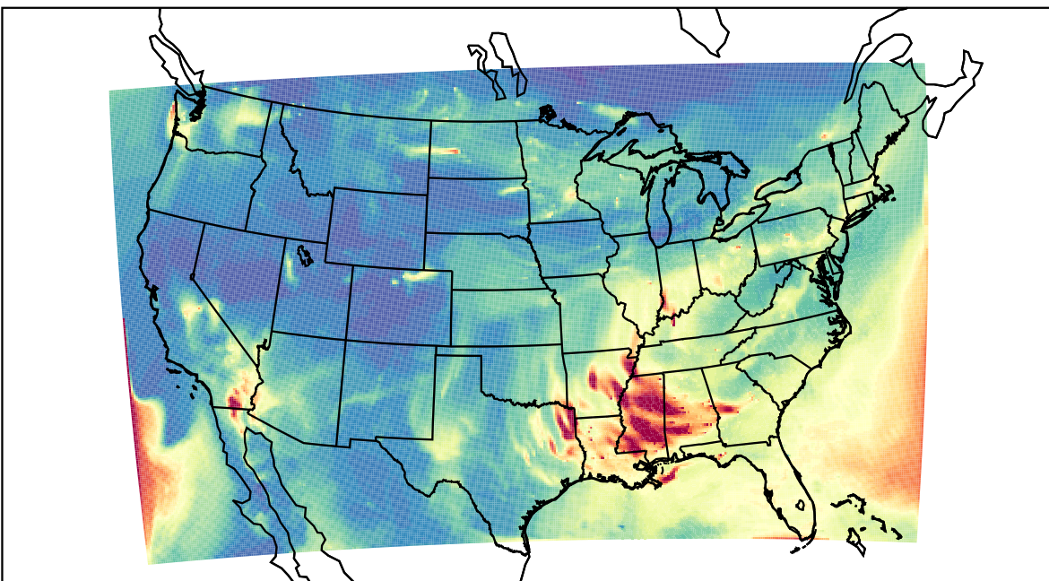
WRF 2020-10-22_08:00:00
