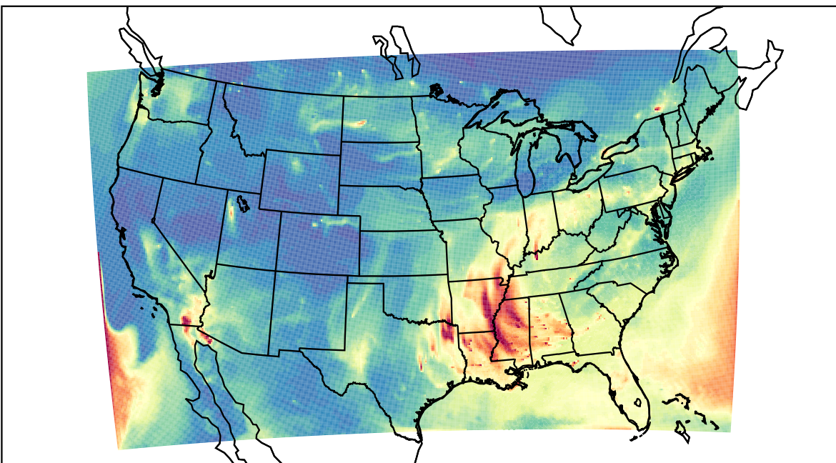
WRF 2020-10-22_12:00:00
