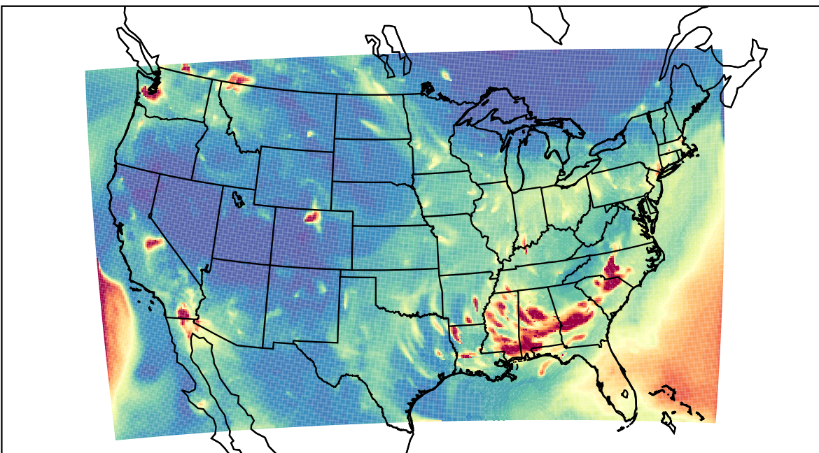
WRF 2020-10-21_05:00:00
