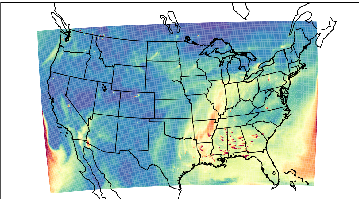
WRF 2020-10-22_20:00:00
