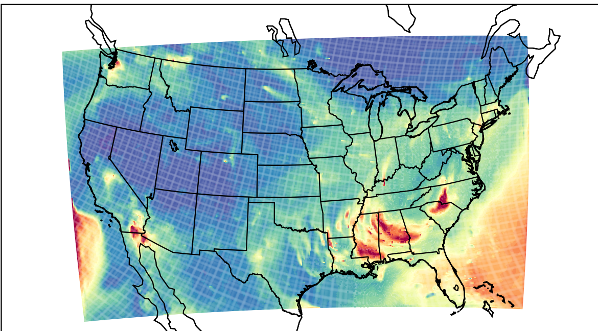
WRF 2020-10-21_09:00:00
