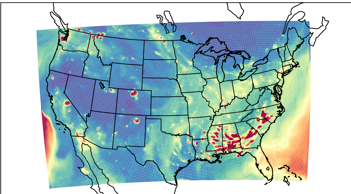
WRF 2020-10-21_02:00:00
