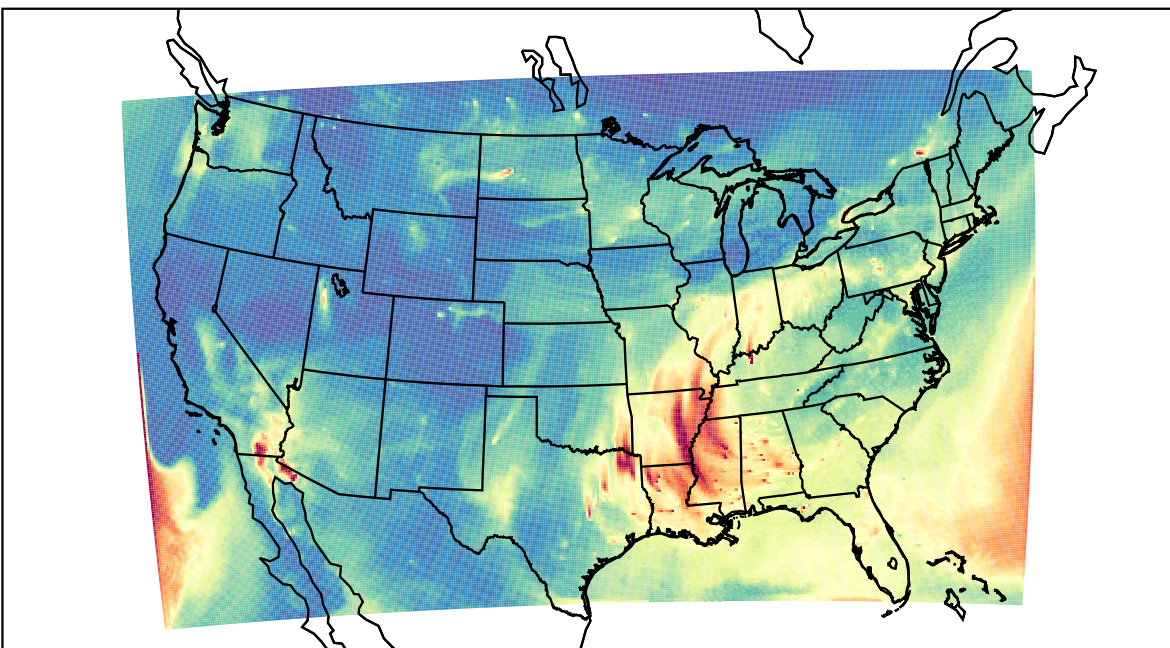
WRF 2020-10-22_13:00:00
