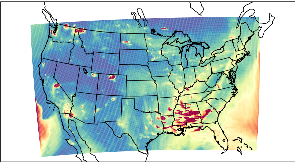
WRF 2020-10-22_02:00:00
