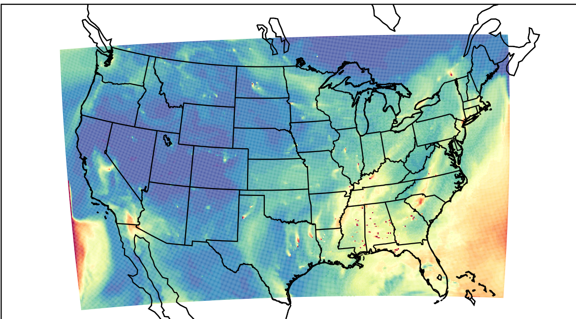
WRF 2020-10-21_17:00:00
