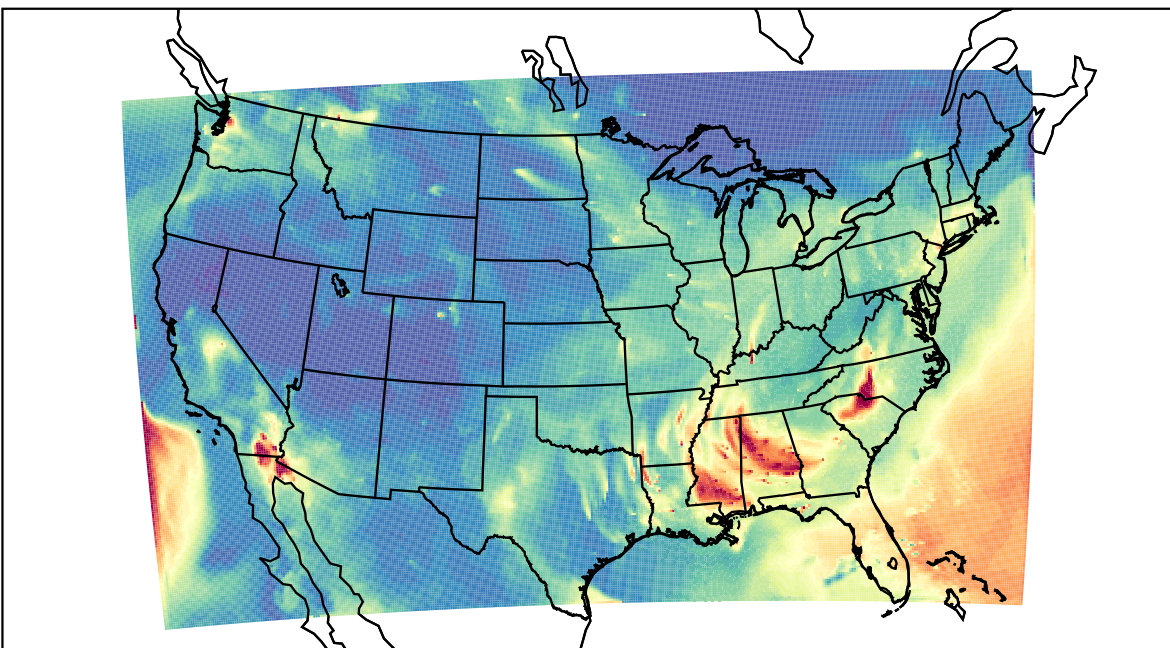
WRF 2020-10-21_10:00:00
