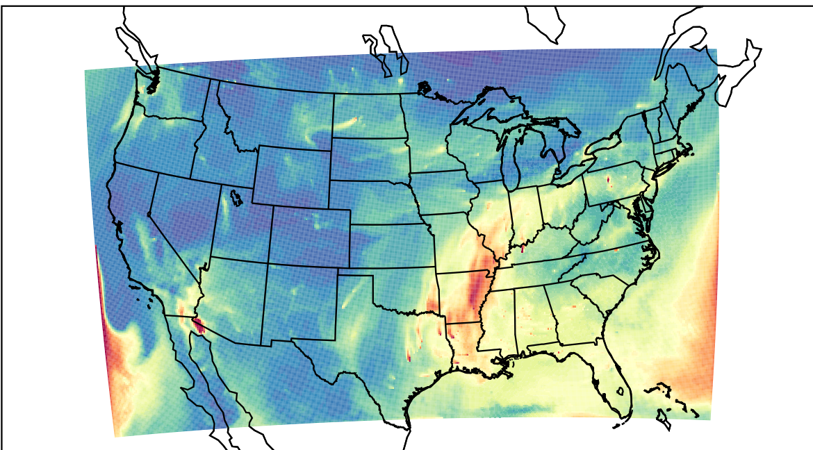
WRF 2020-10-22_16:00:00
