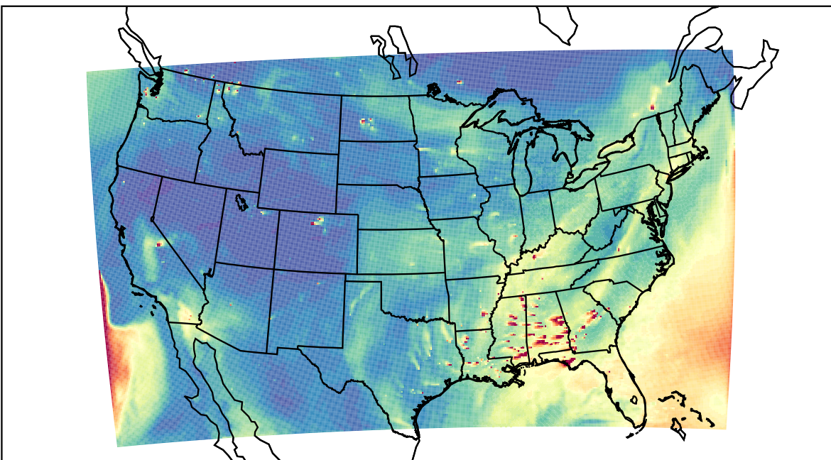
WRF 2020-10-21_21:00:00
