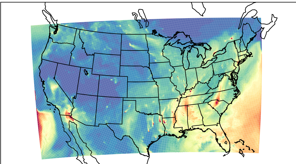
WRF 2020-10-21_15:00:00
