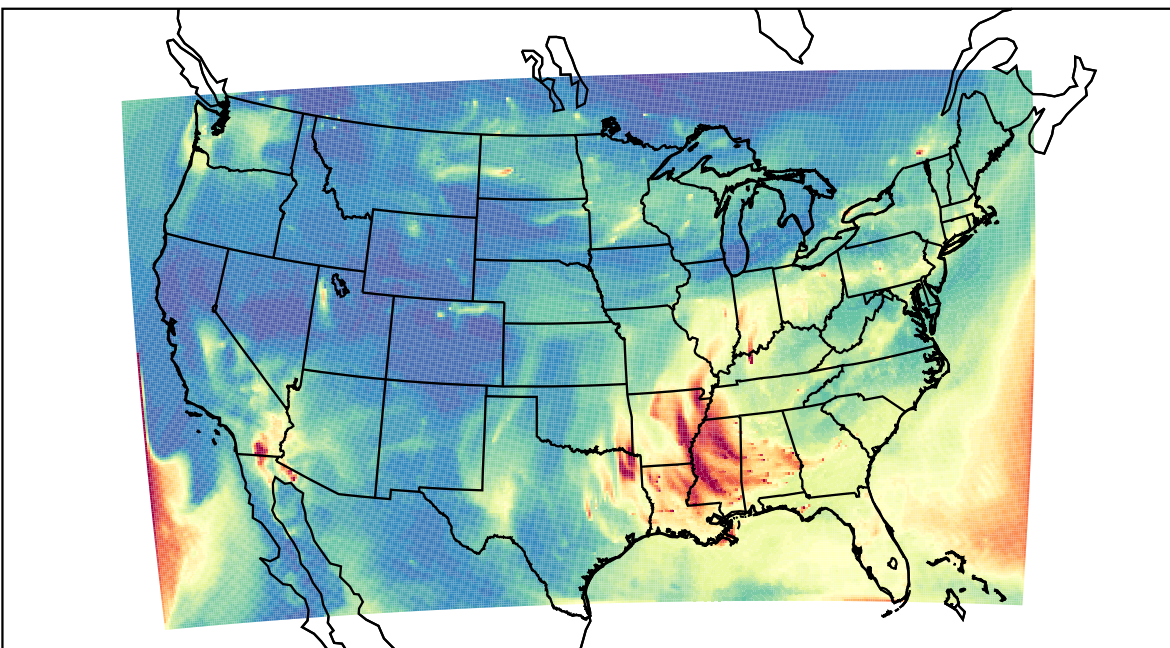
WRF 2020-10-22_11:00:00
