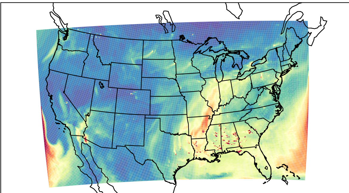
WRF 2020-10-22_19:00:00
