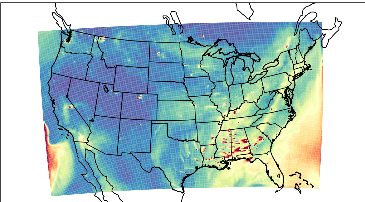
WRF 2020-10-21_22:00:00
