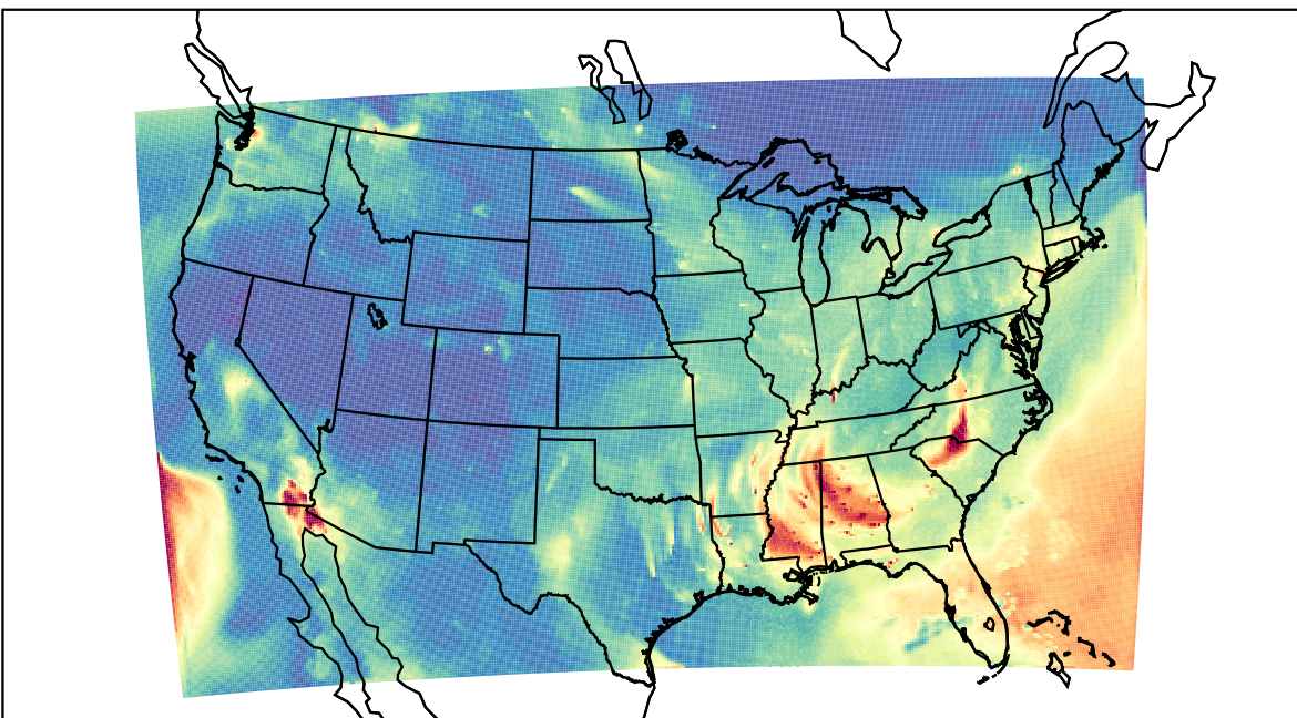
WRF 2020-10-21_11:00:00
