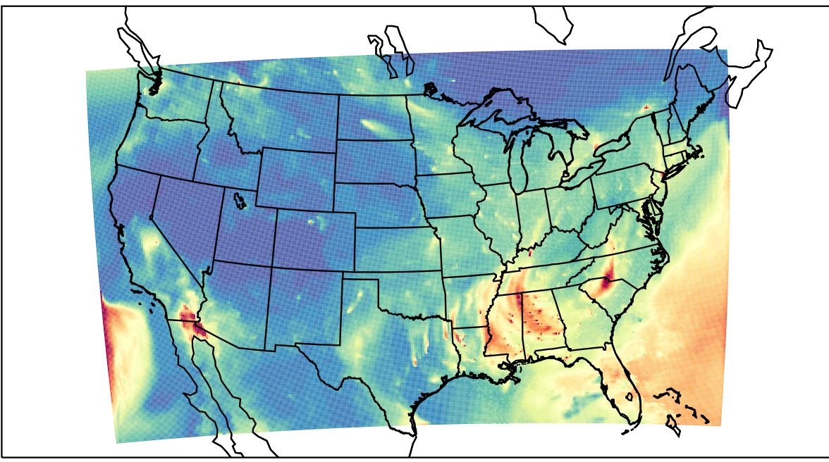
WRF 2020-10-21_13:00:00
