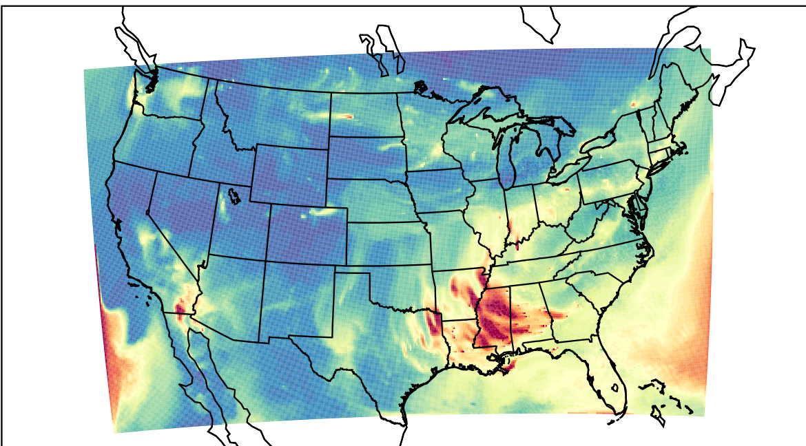
WRF 2020-10-22_09:00:00
