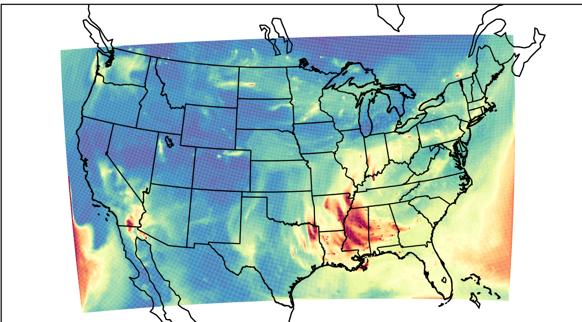
WRF 2020-10-22_10:00:00
