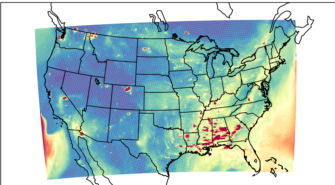
WRF 2020-10-22_00:00:00
