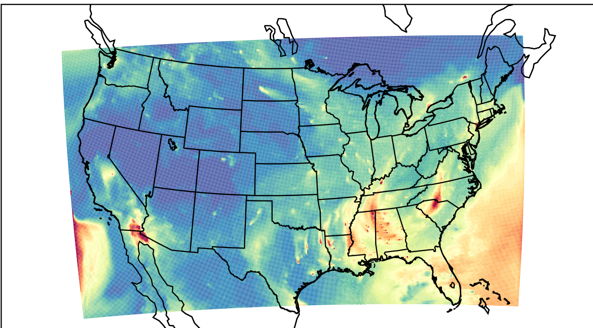
WRF 2020-10-21_14:00:00
