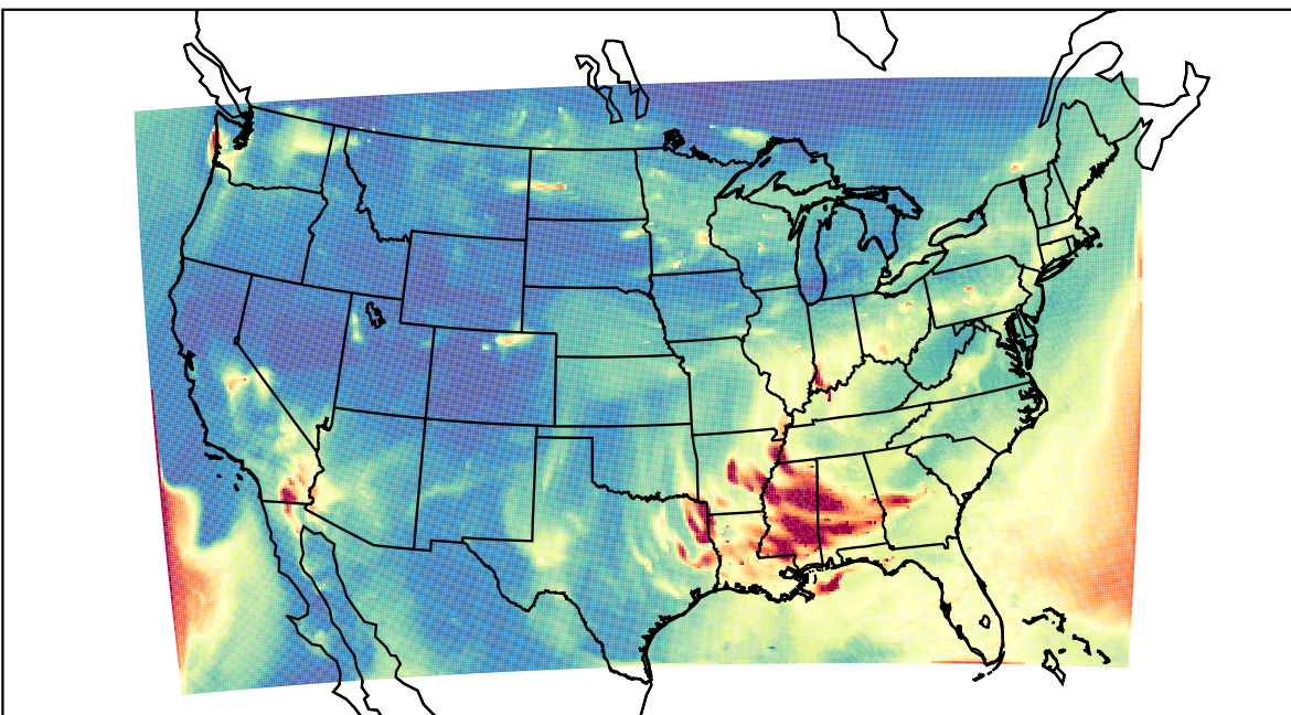
WRF 2020-10-22_07:00:00
