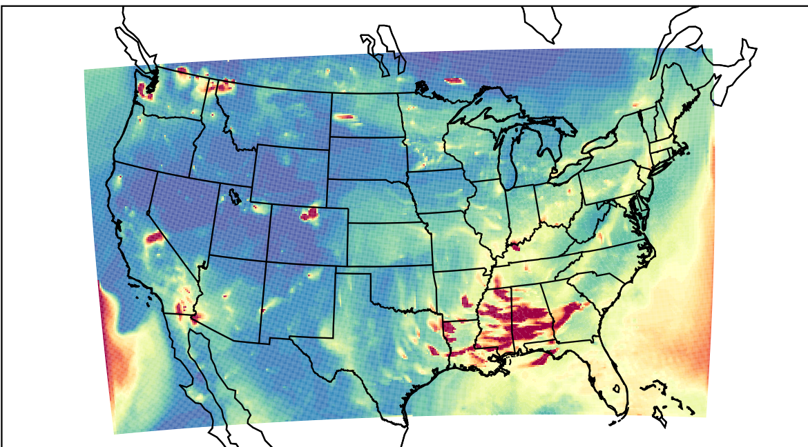
WRF 2020-10-22_03:00:00
