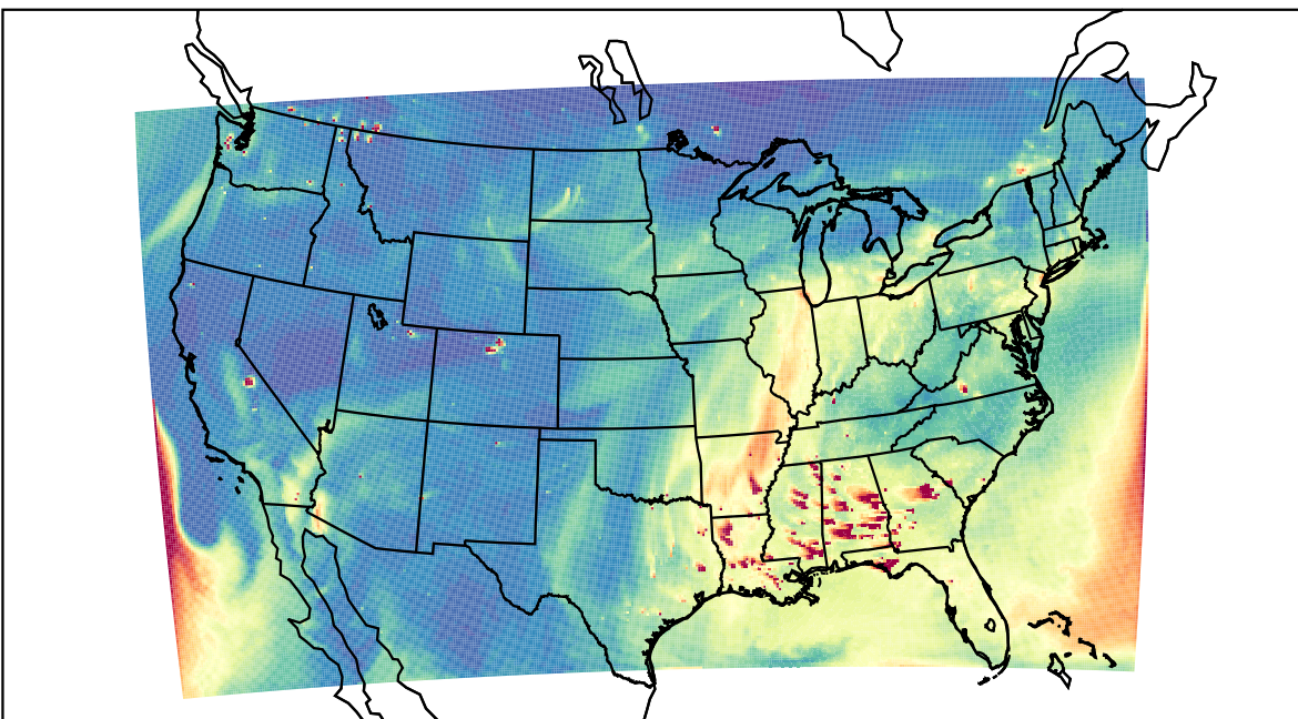
WRF 2020-10-22_22:00:00
