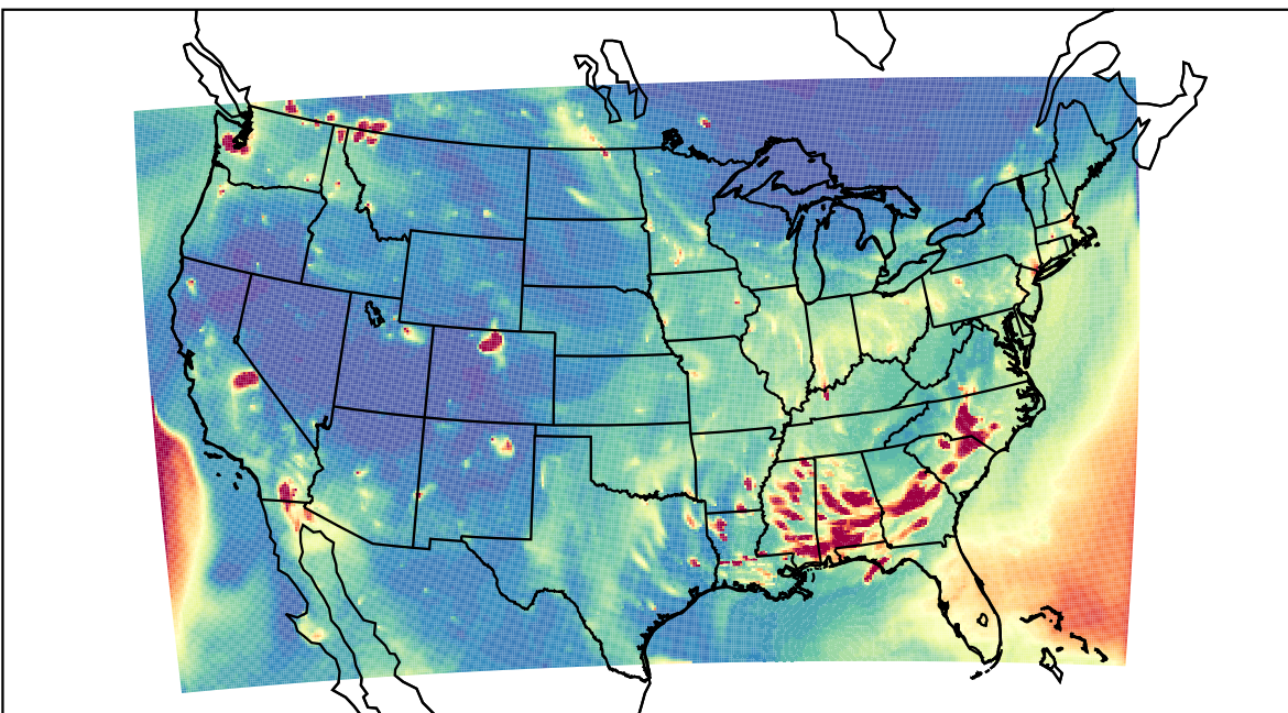
WRF 2020-10-21_03:00:00
