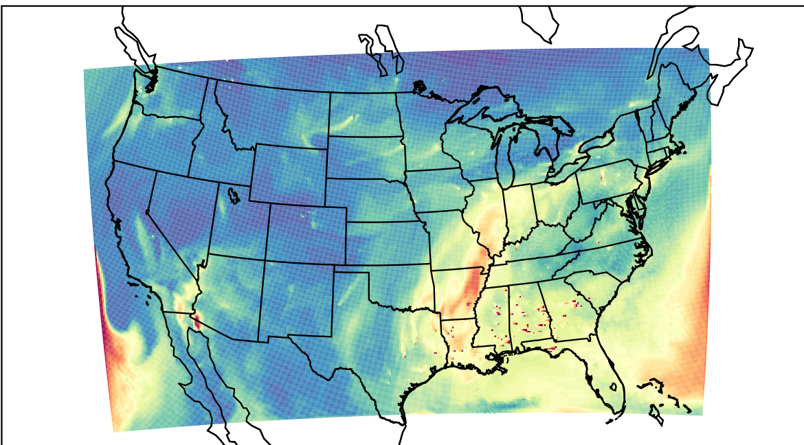
WRF 2020-10-22_18:00:00
