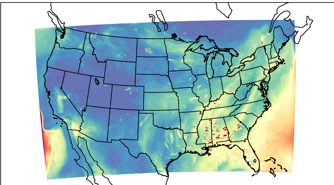
WRF 2020-10-21_20:00:00
