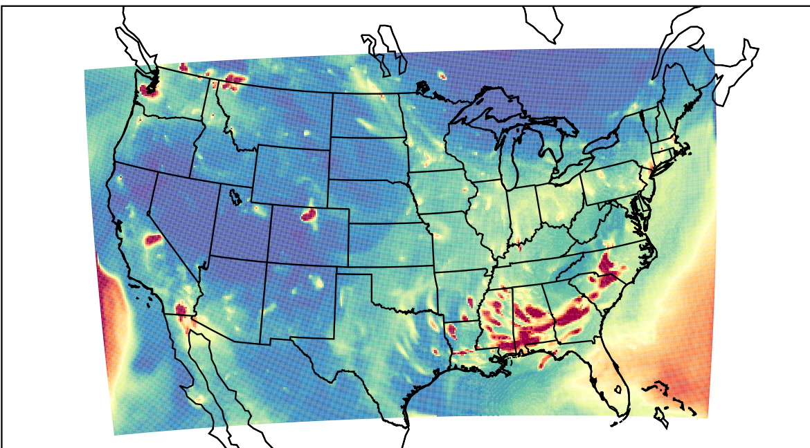
WRF 2020-10-21_04:00:00
