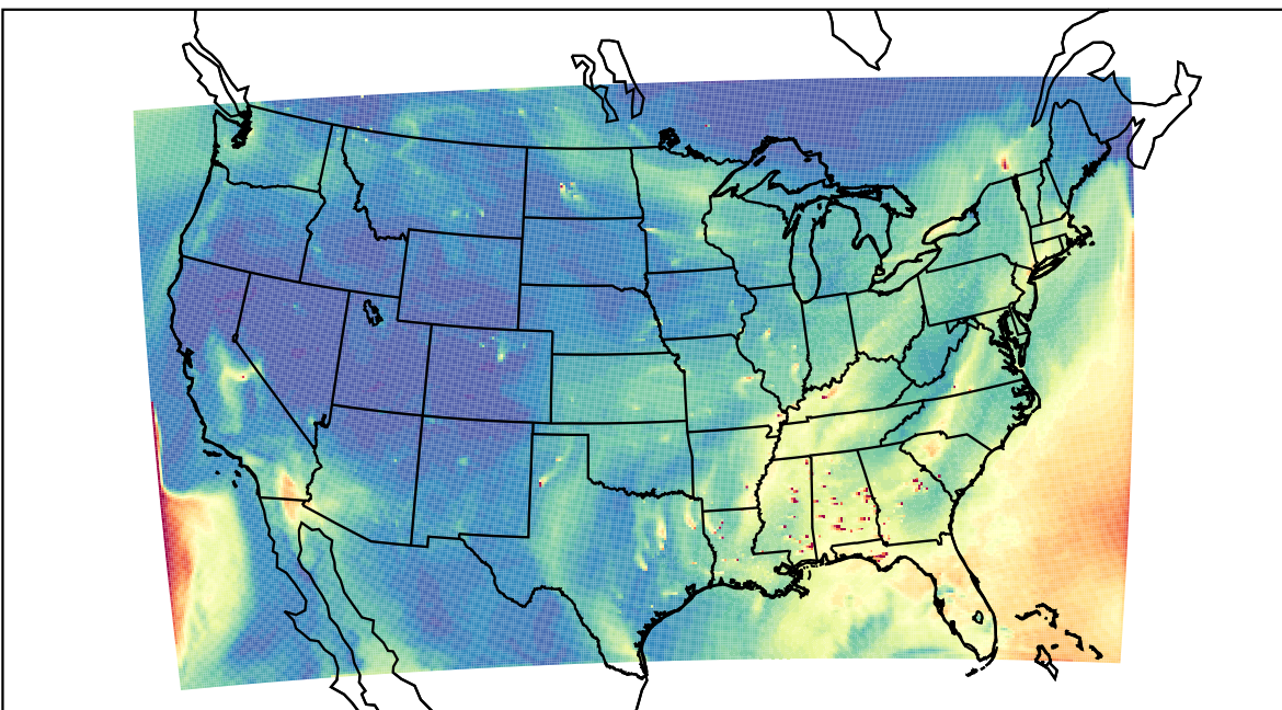
WRF 2020-10-21_18:00:00
