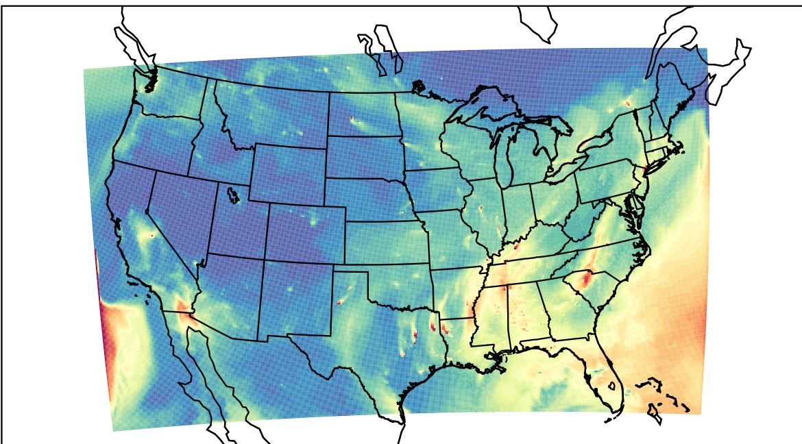
WRF 2020-10-21_16:00:00
