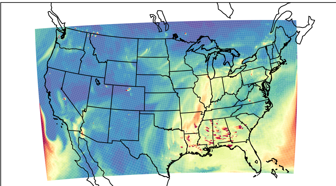
WRF 2020-10-22_21:00:00
