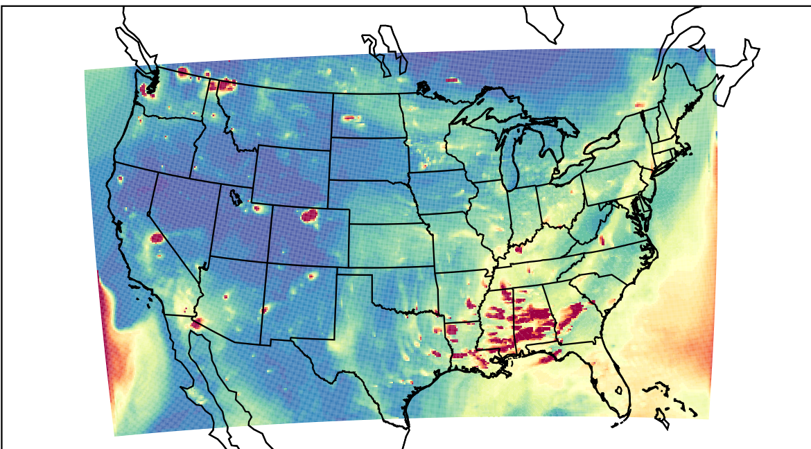
WRF 2020-10-22_01:00:00
