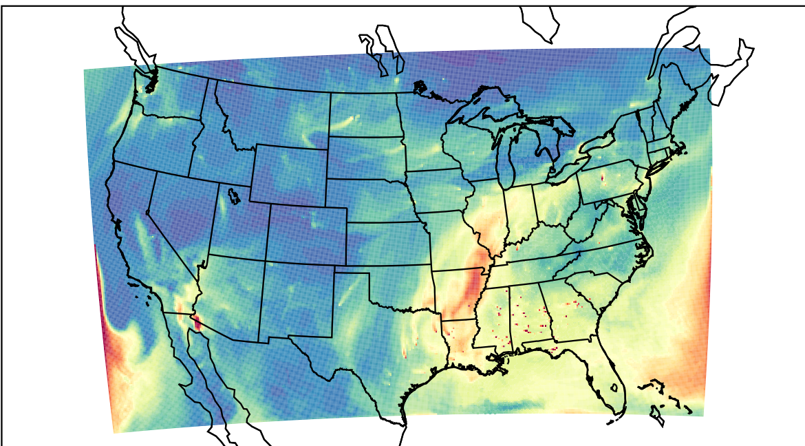
WRF 2020-10-22_17:00:00
