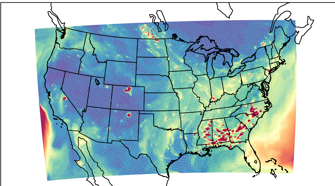
WRF 2020-10-21_00:00:00
