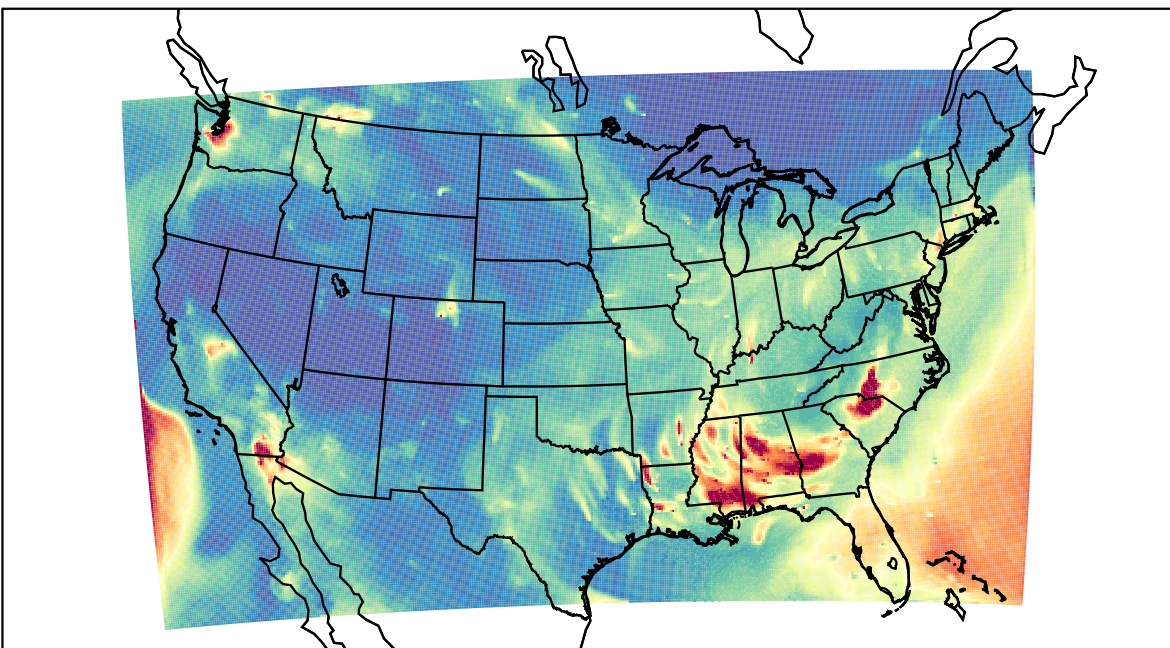
WRF 2020-10-21_07:00:00
