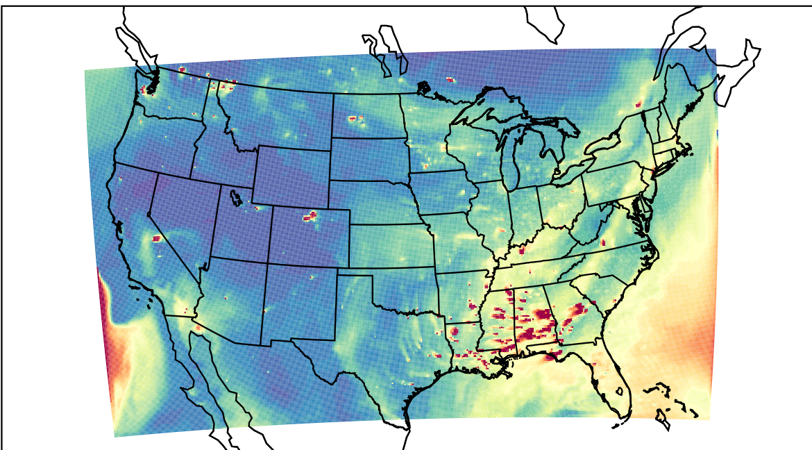
WRF 2020-10-21_23:00:00
