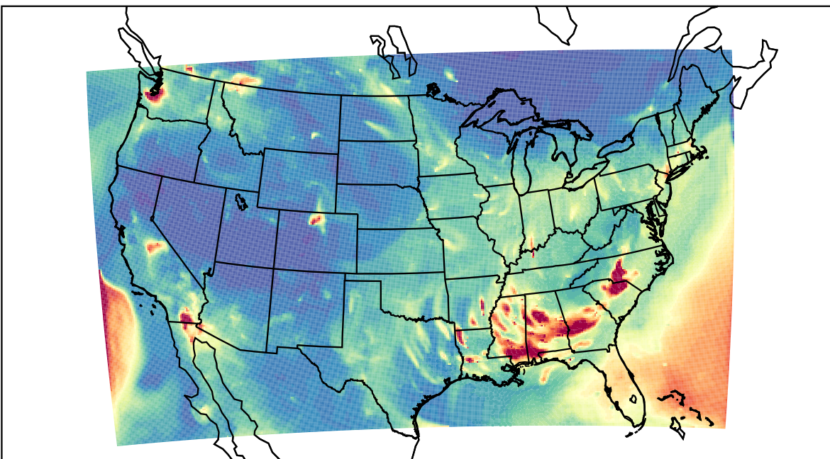
WRF 2020-10-21_06:00:00
