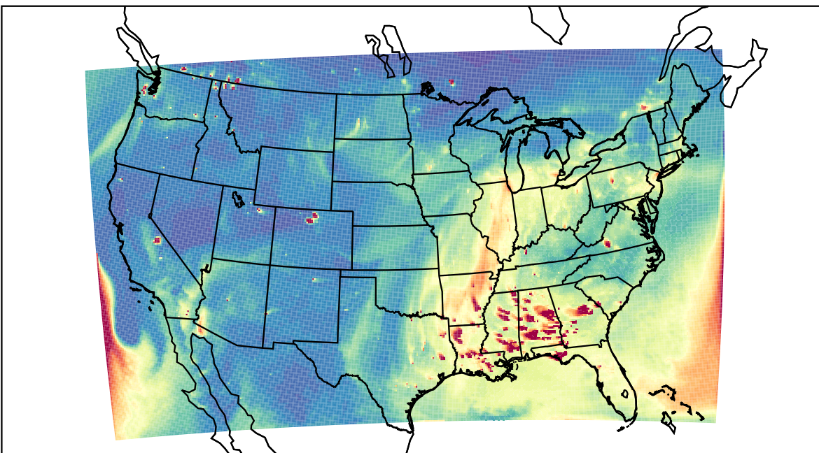
WRF 2020-10-22_23:00:00
