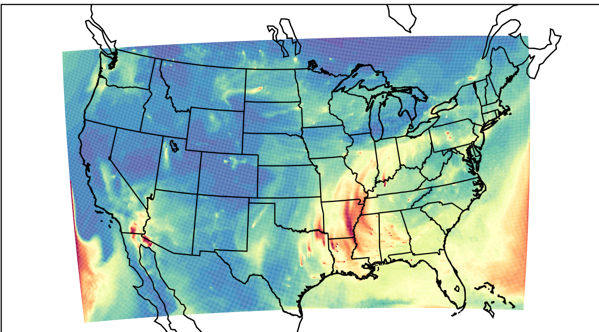
WRF 2020-10-22_14:00:00
