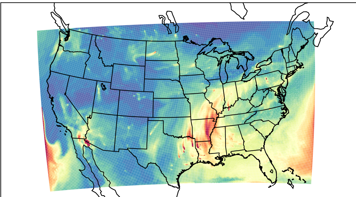
WRF 2020-10-22_15:00:00
