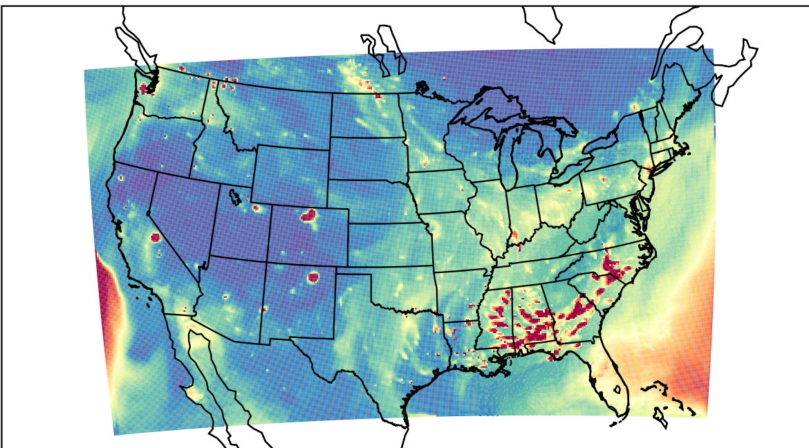
WRF 2020-10-21_01:00:00
