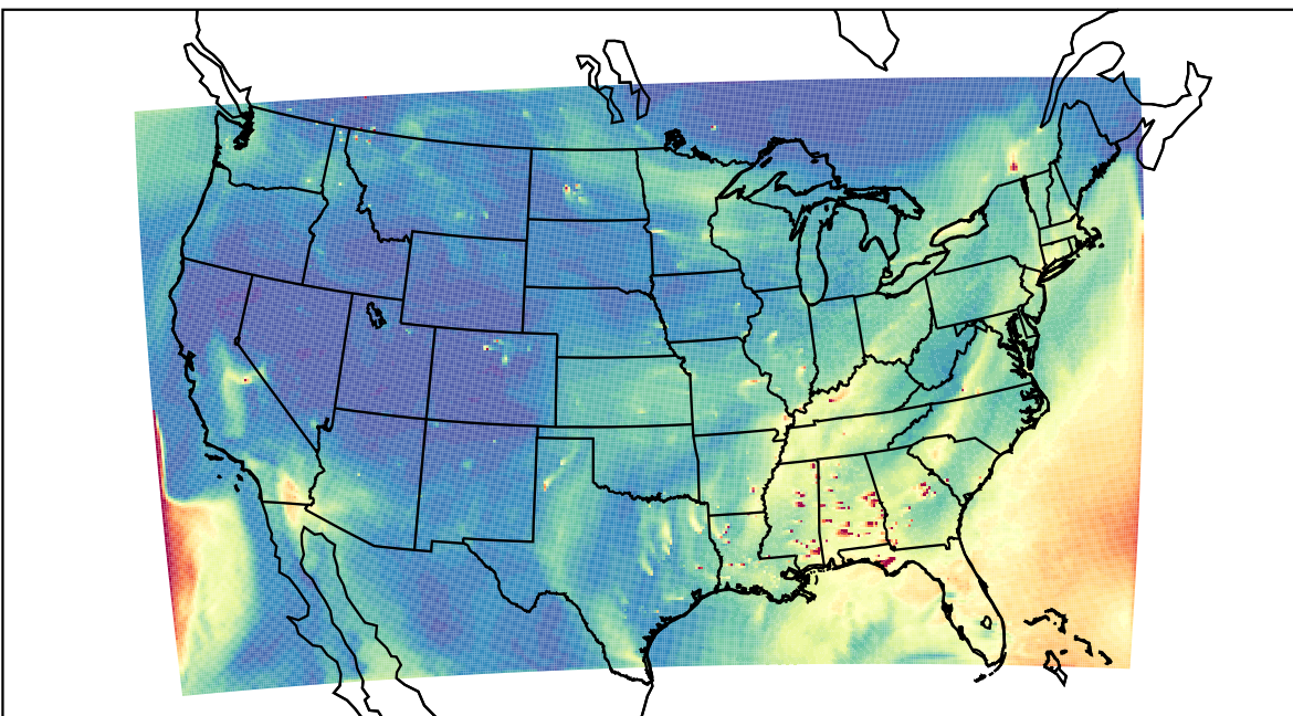
WRF 2020-10-21_19:00:00
