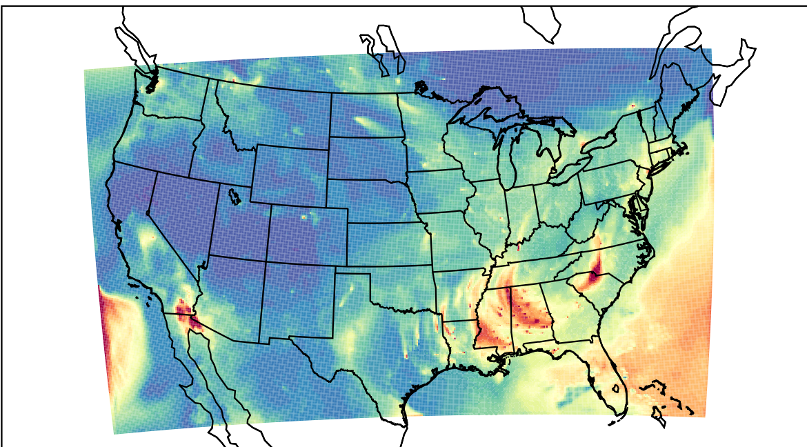
WRF 2020-10-21_12:00:00
