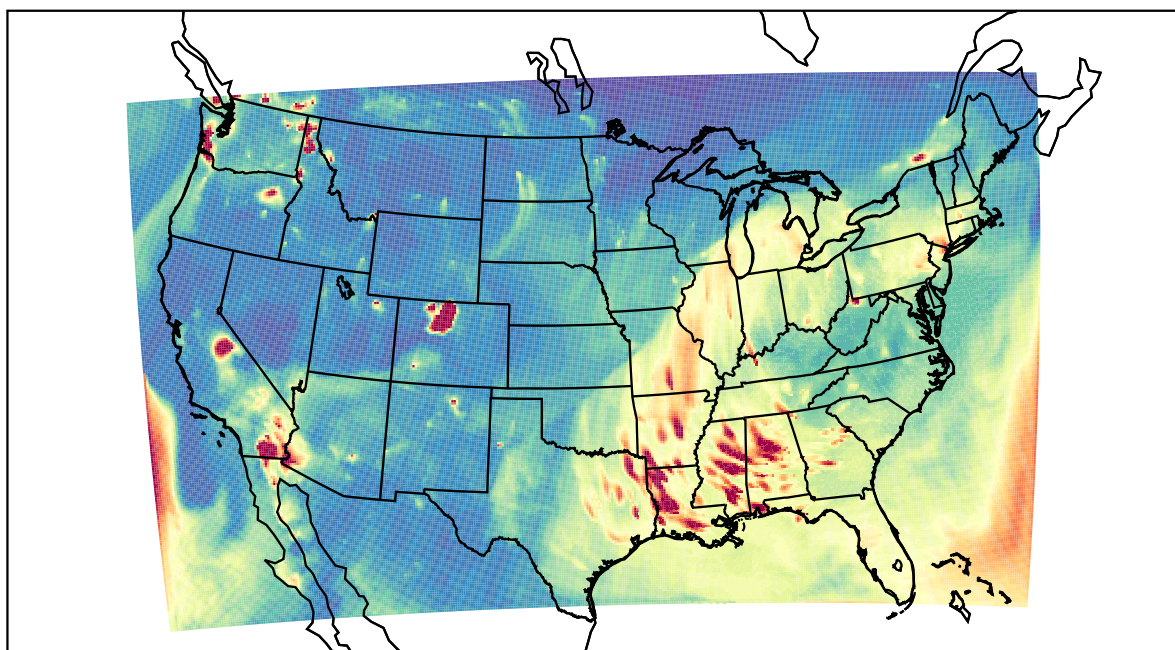
WRF 2020-10-23_04:00:00
