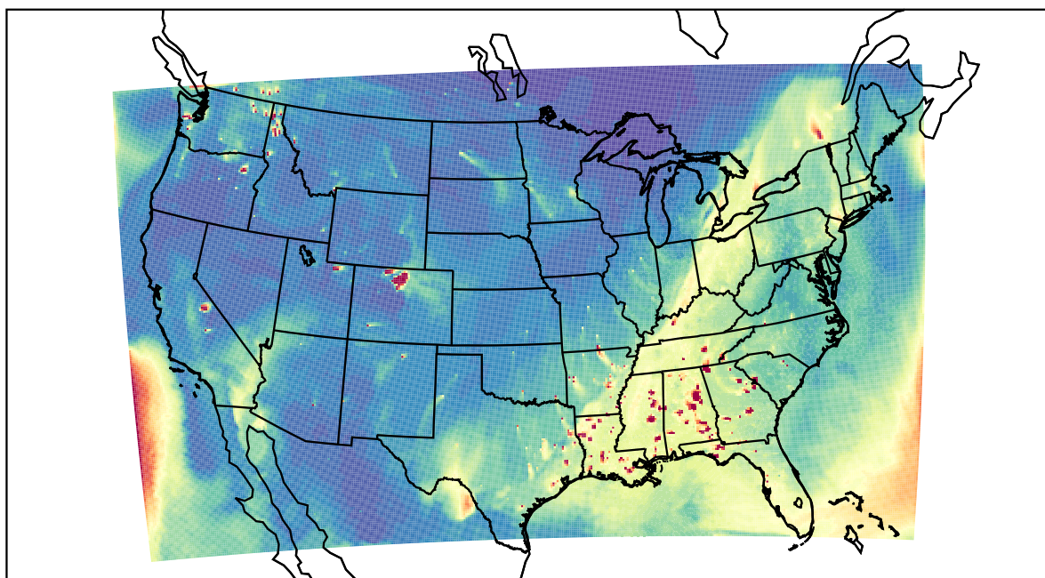
WRF 2020-10-23_22:00:00
