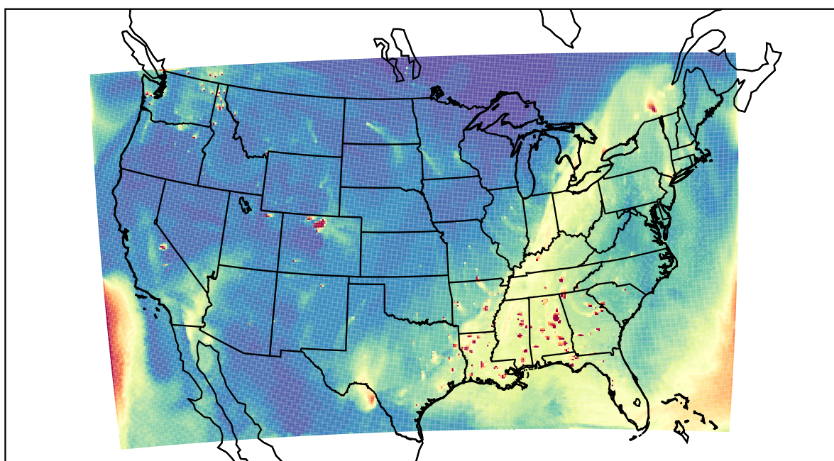
WRF 2020-10-23_21:00:00
