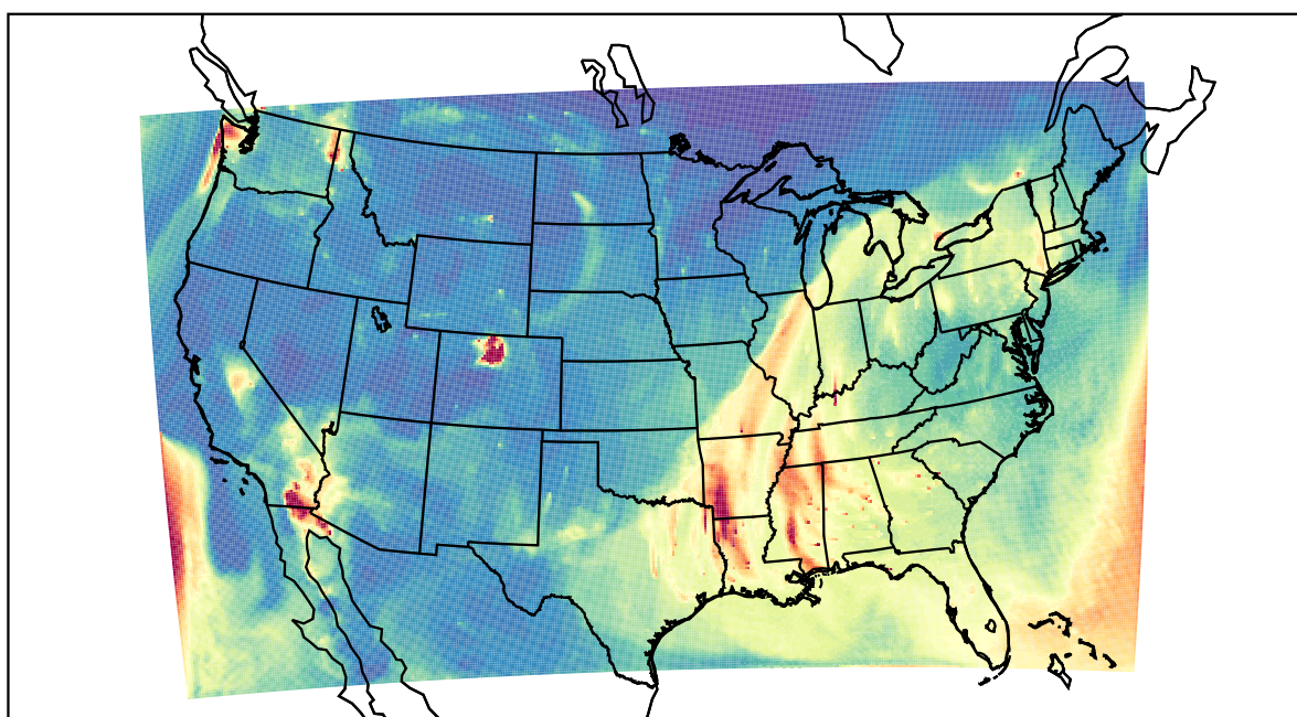
WRF 2020-10-23_10:00:00
