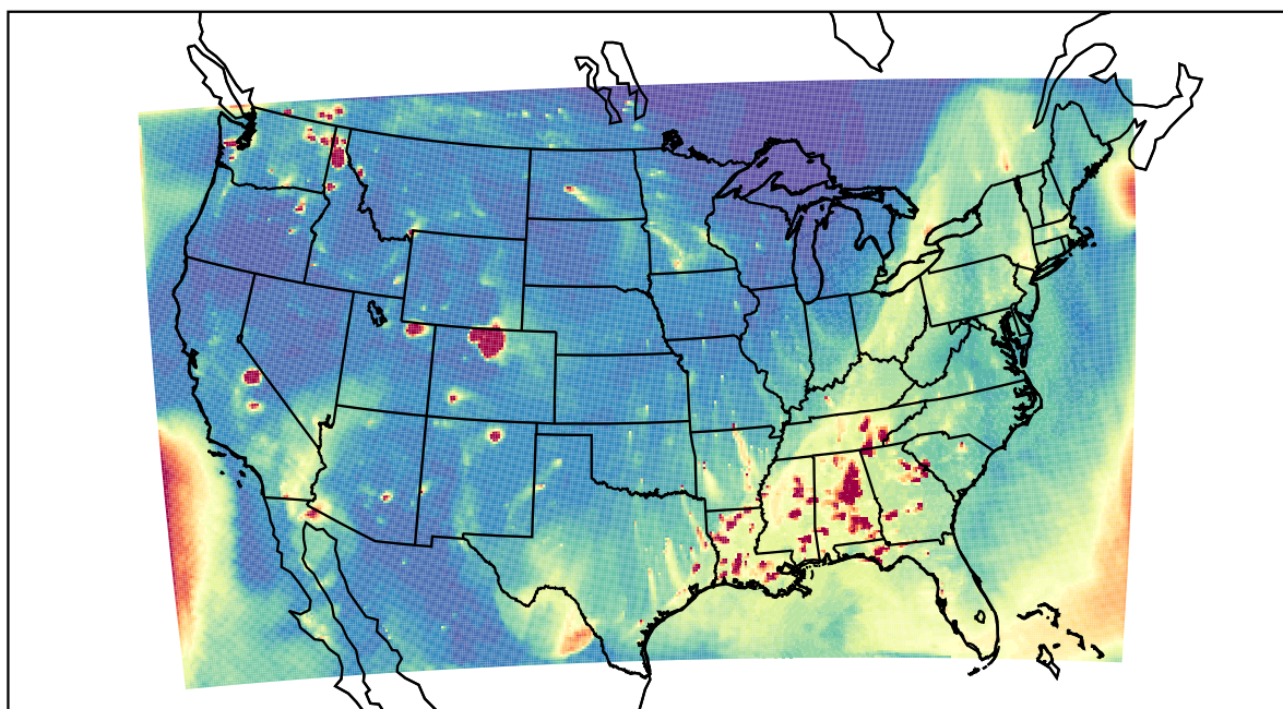
WRF 2020-10-24_01:00:00
