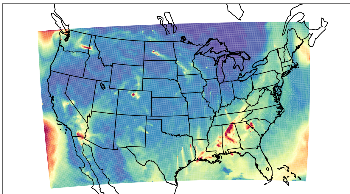
WRF 2020-10-24_08:00:00
