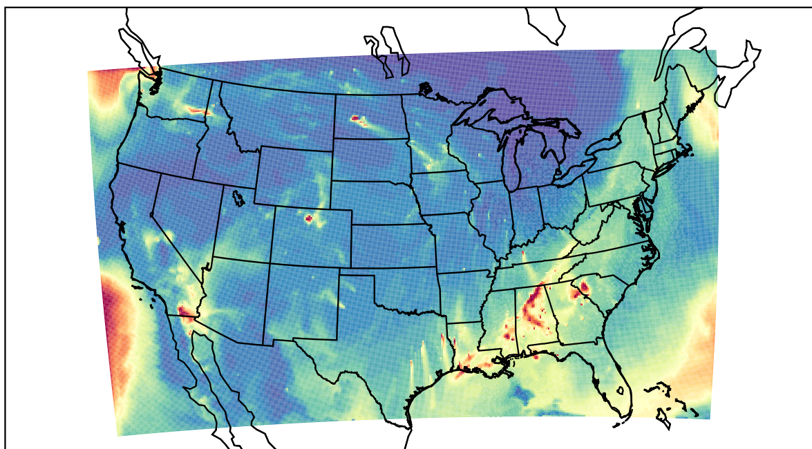
WRF 2020-10-24_09:00:00
