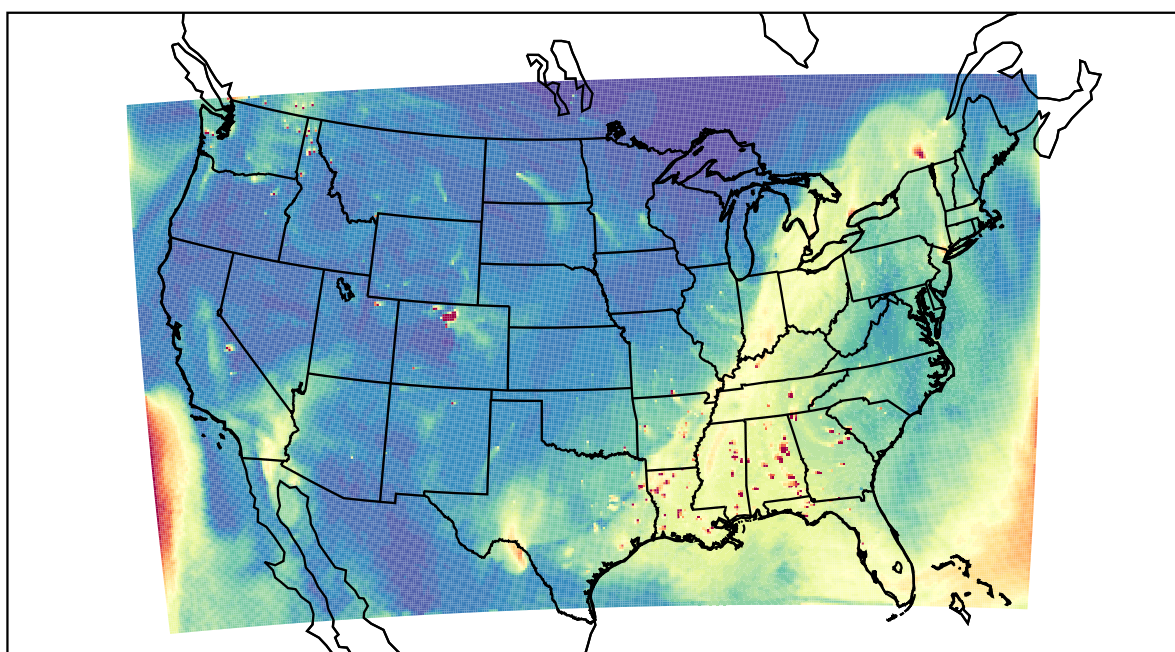
WRF 2020-10-23_20:00:00
