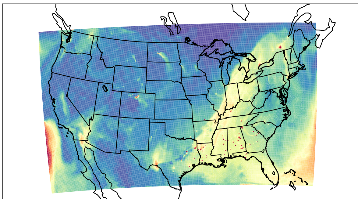
WRF 2020-10-23_18:00:00
