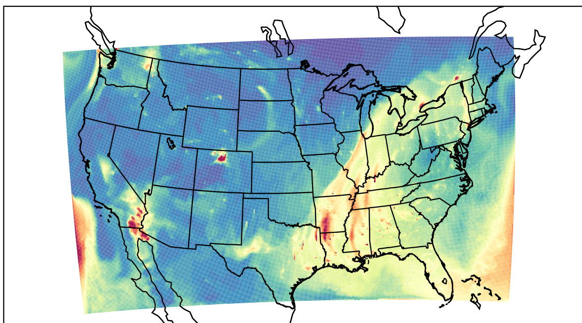
WRF 2020-10-23_13:00:00
