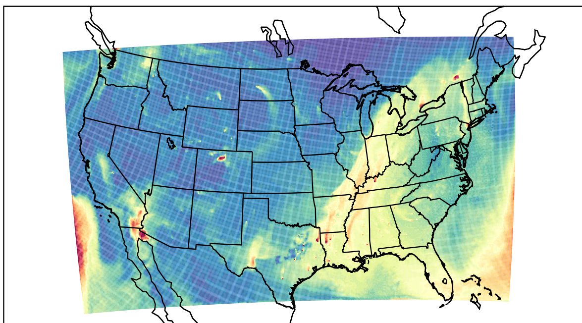
WRF 2020-10-23_16:00:00
