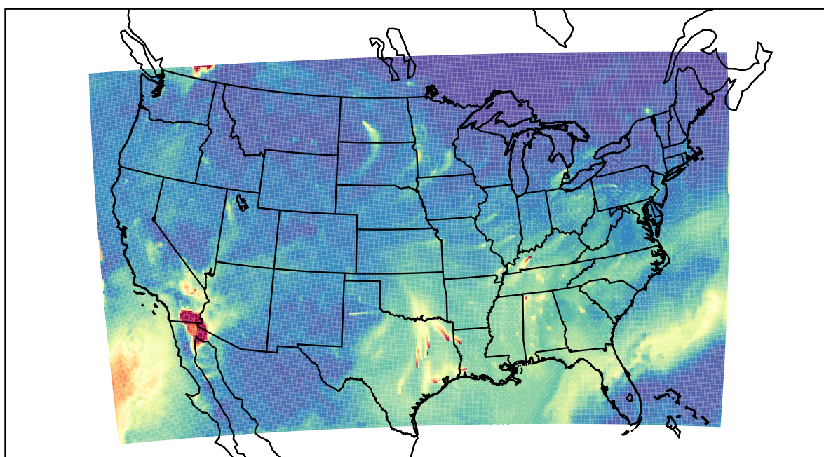
WRF 2020-10-25_16:00:00
