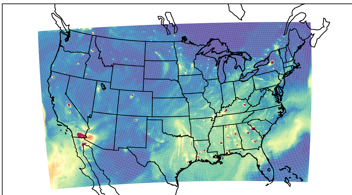
WRF 2020-10-25_23:00:00
