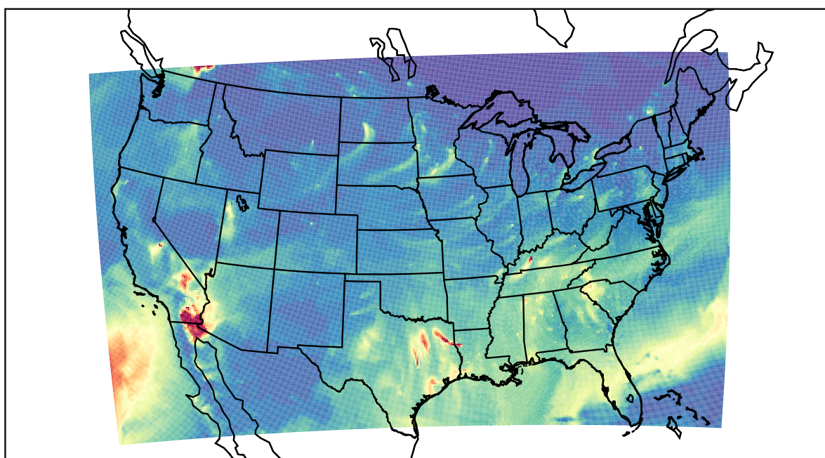
WRF 2020-10-25_10:00:00
