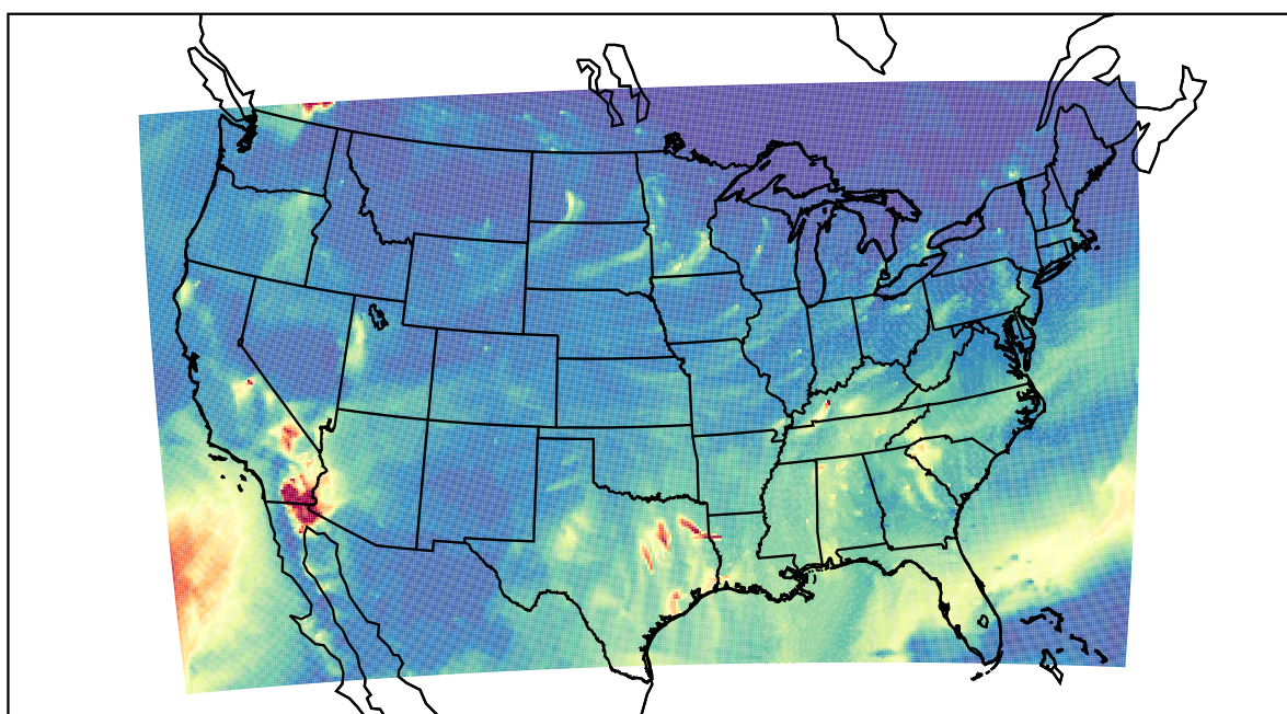
WRF 2020-10-25_09:00:00
