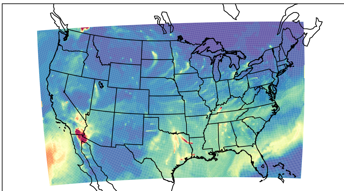
WRF 2020-10-25_14:00:00
