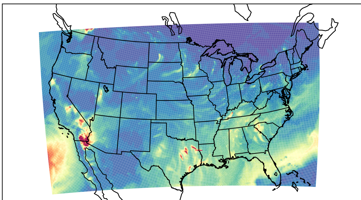
WRF 2020-10-25_08:00:00
