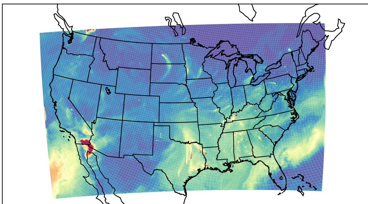
WRF 2020-10-25_18:00:00
