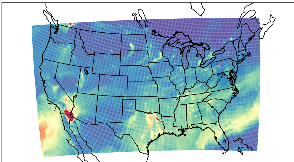
WRF 2020-10-25_13:00:00
