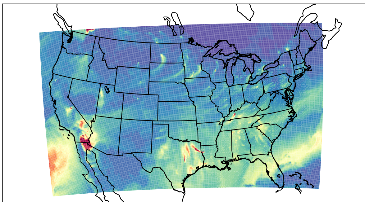
WRF 2020-10-25_11:00:00
