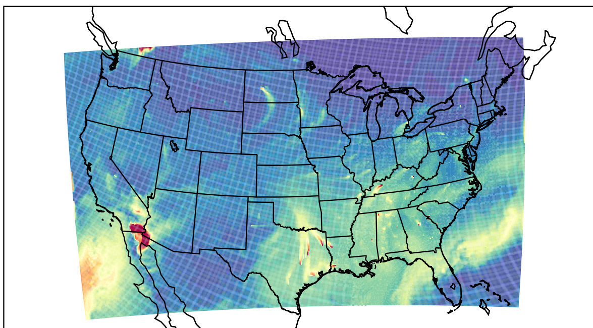
WRF 2020-10-25_17:00:00
