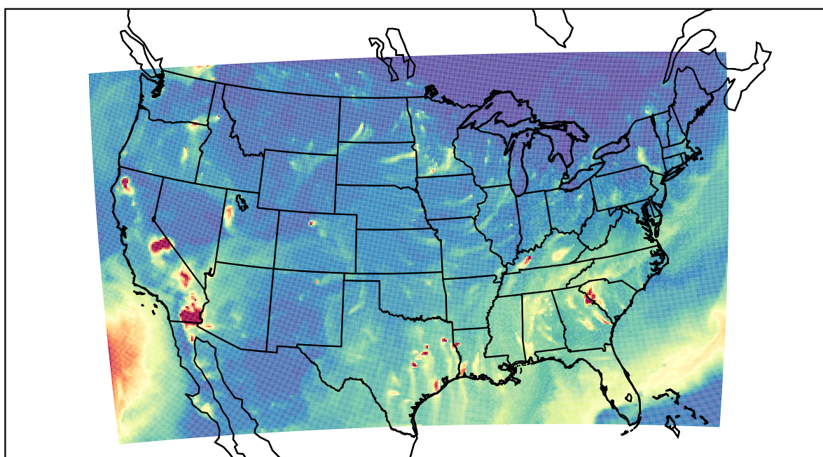
WRF 2020-10-25_04:00:00
