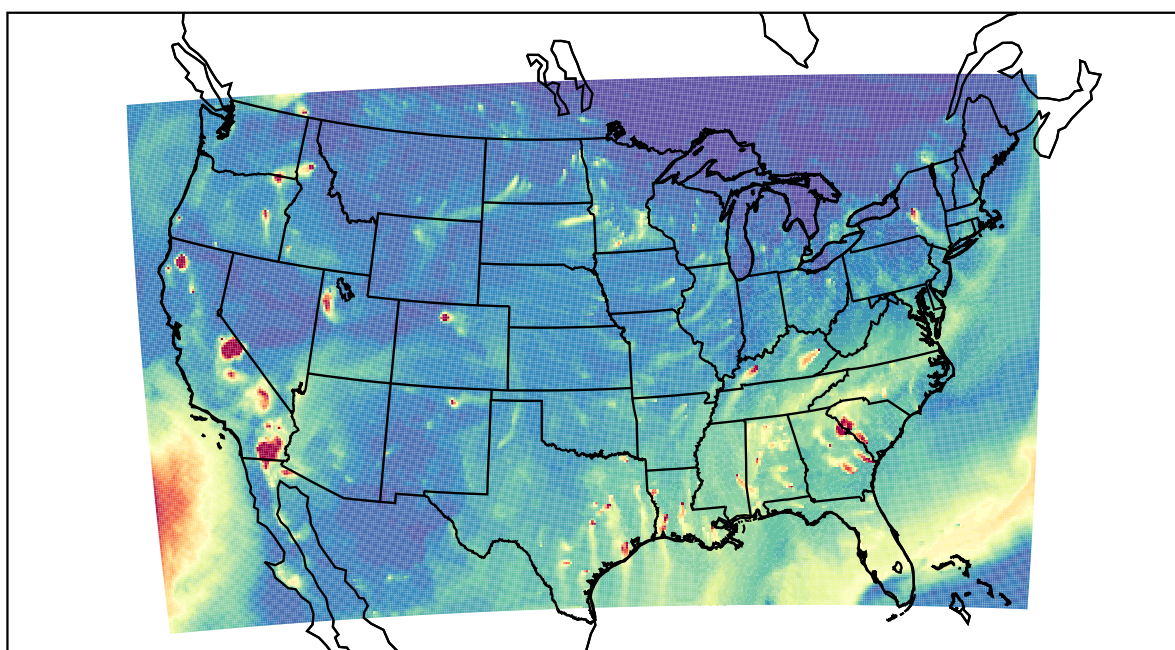
WRF 2020-10-25_02:00:00
