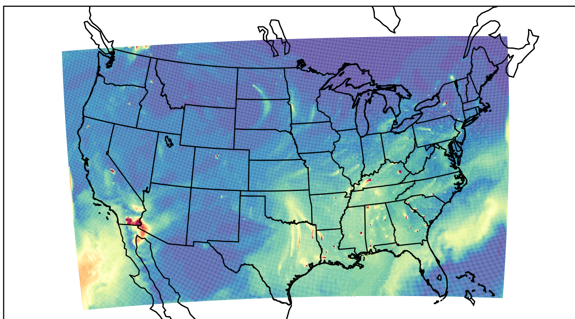
WRF 2020-10-25_20:00:00
