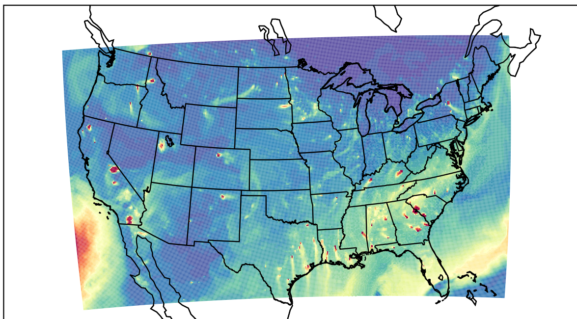
WRF 2020-10-25_00:00:00
