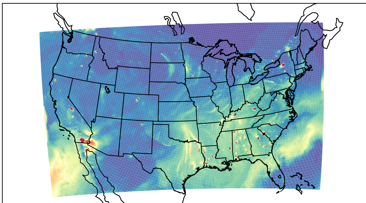
WRF 2020-10-25_22:00:00
