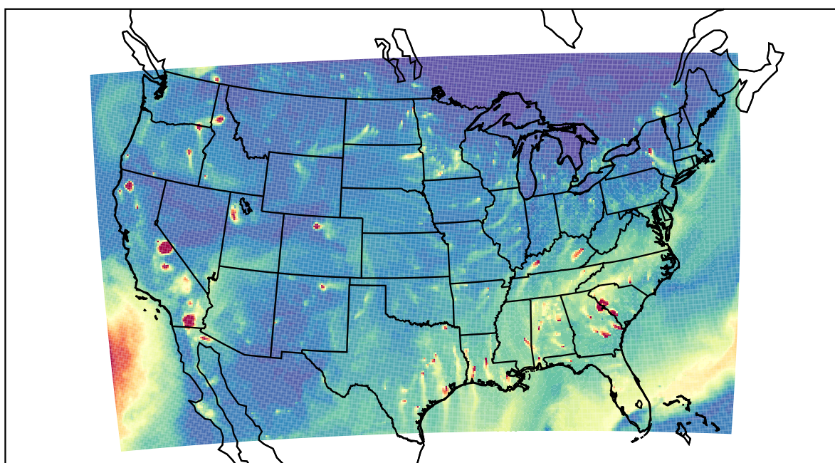
WRF 2020-10-25_01:00:00
