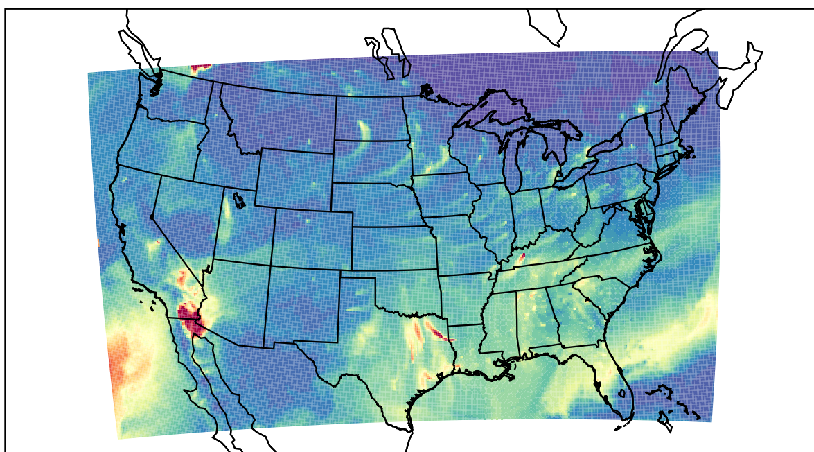
WRF 2020-10-25_12:00:00
