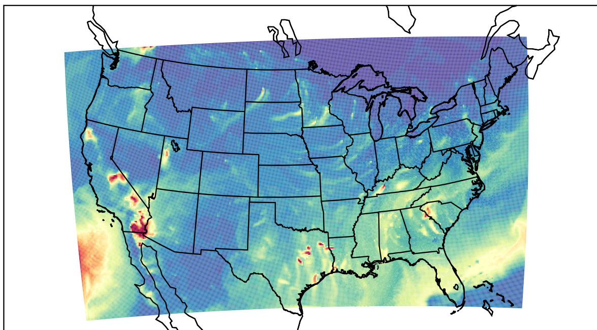
WRF 2020-10-25_06:00:00
