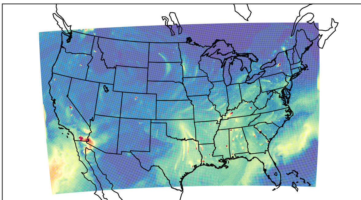
WRF 2020-10-25_21:00:00
