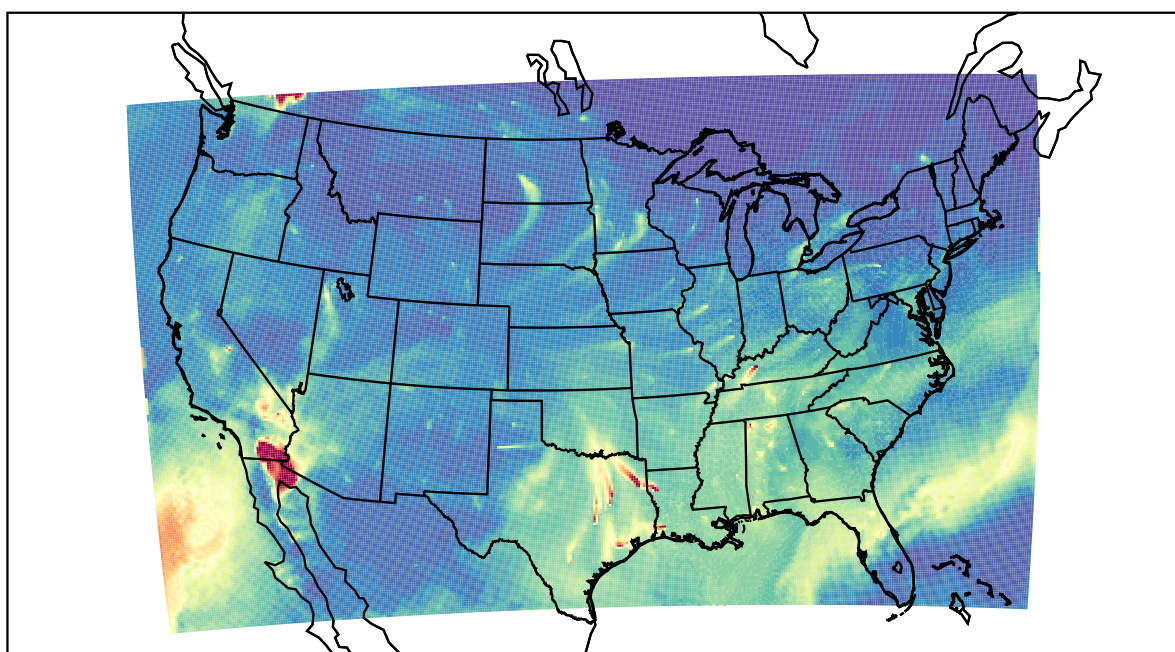
WRF 2020-10-25_15:00:00
