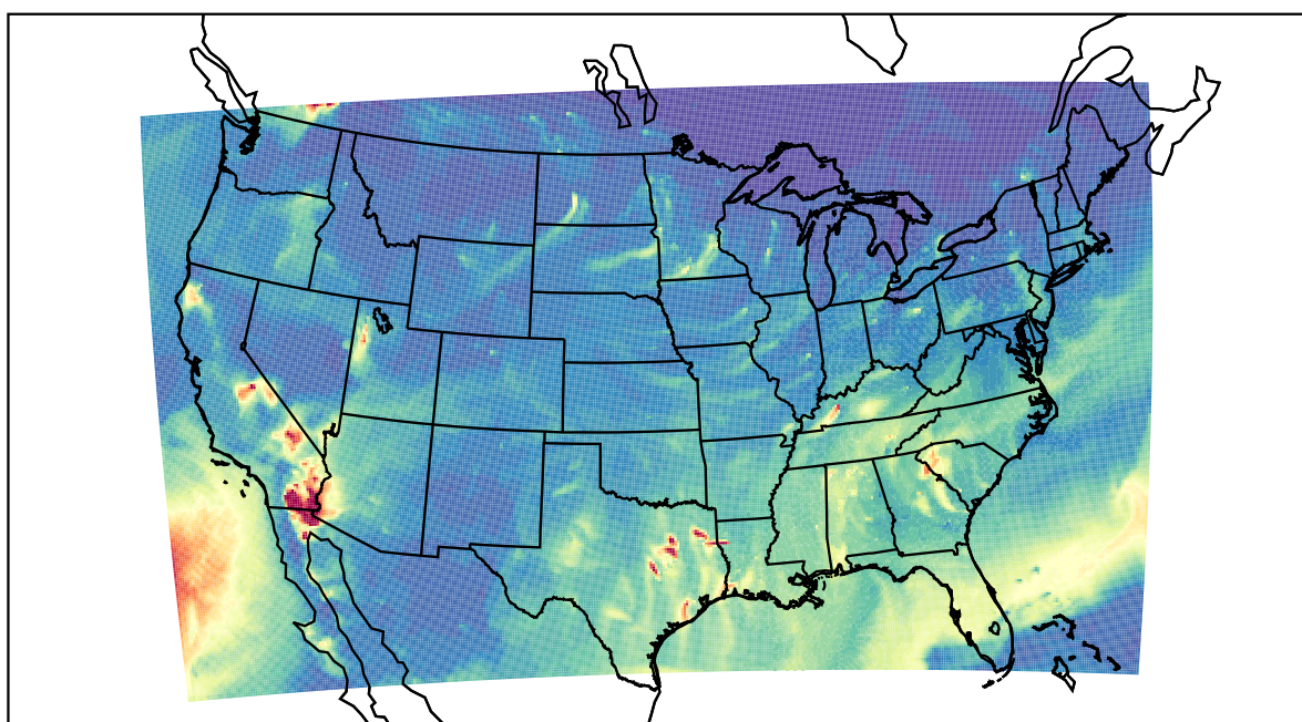
WRF 2020-10-25_07:00:00
