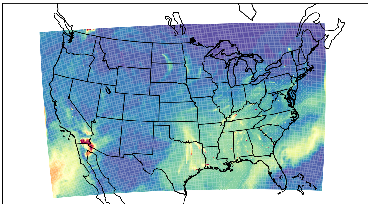
WRF 2020-10-25_19:00:00
