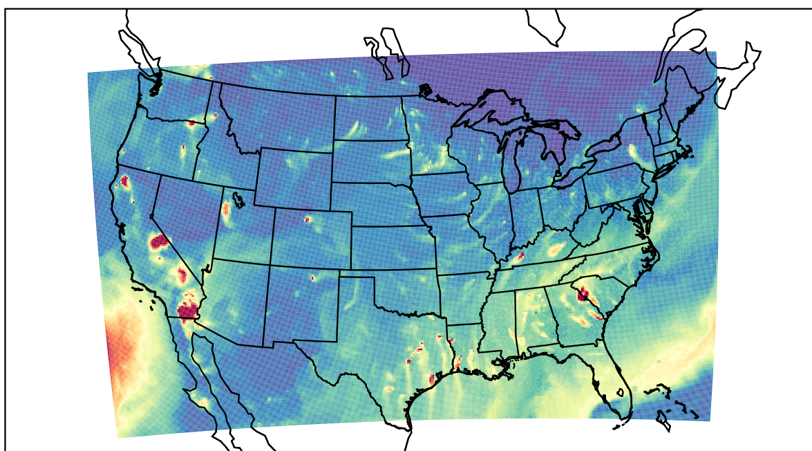
WRF 2020-10-25_03:00:00
