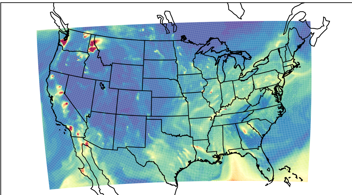
WRF 2020-10-29_04:00:00
