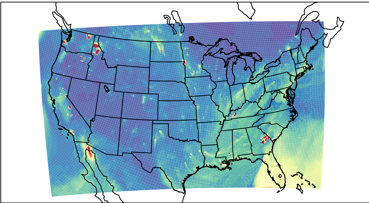
WRF 2020-10-29_23:00:00
