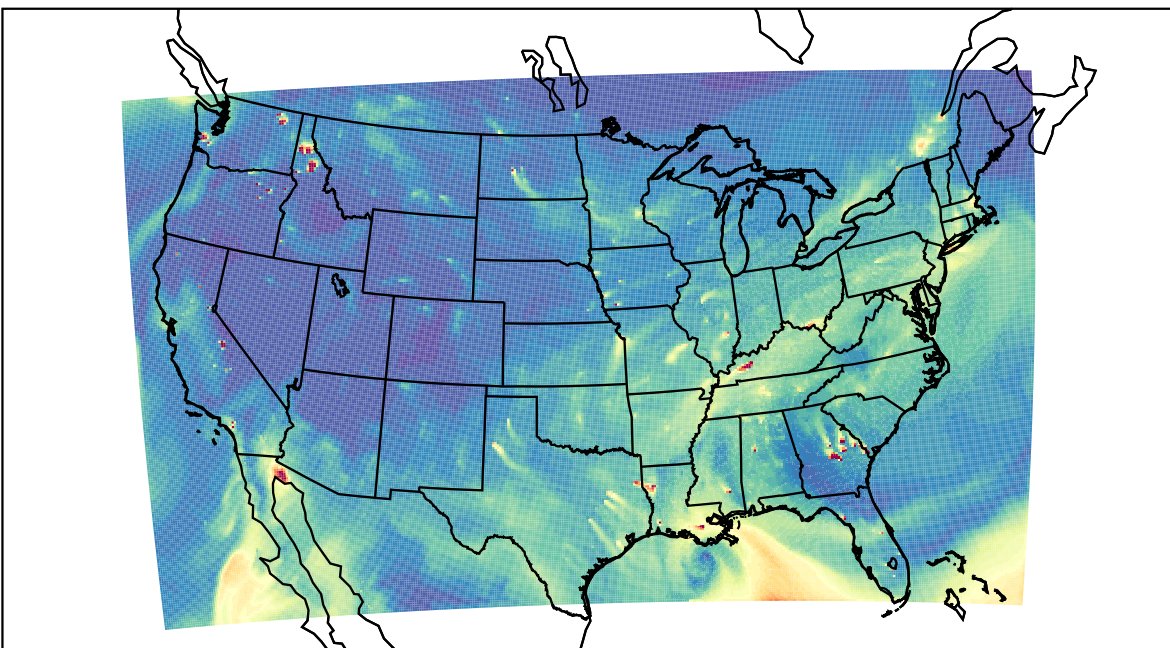
WRF 2020-10-28_21:00:00
