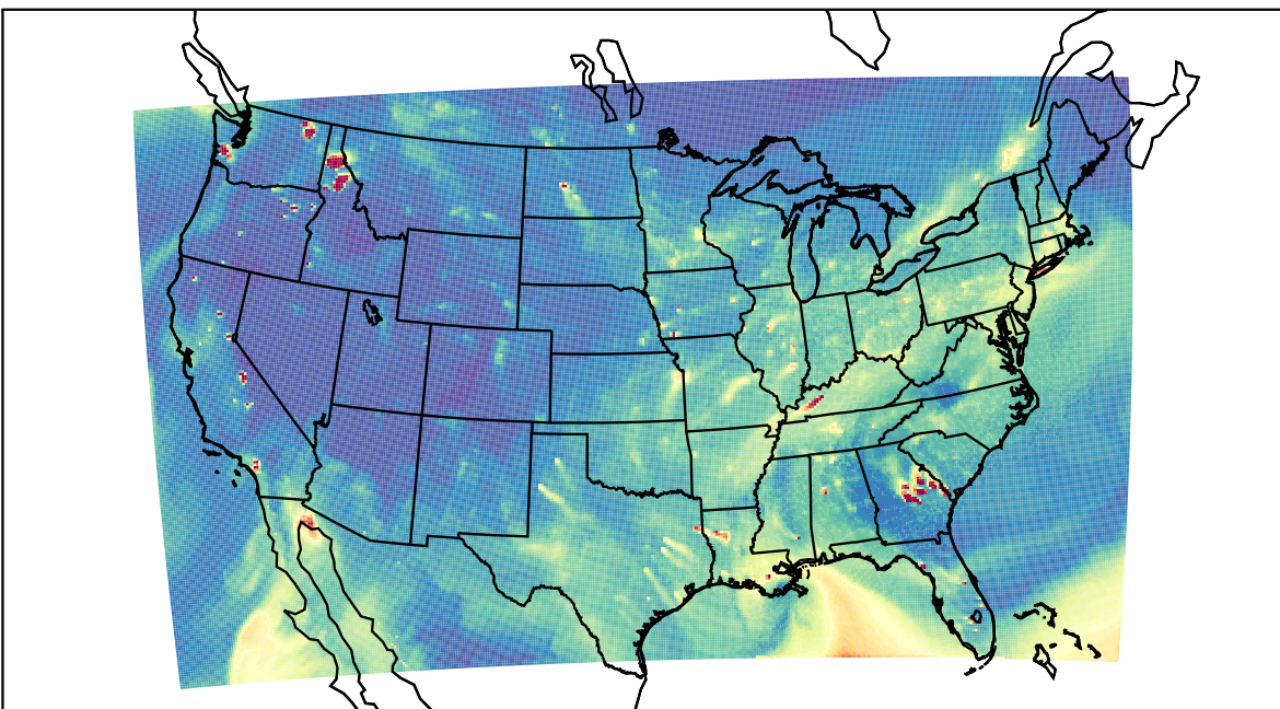
WRF 2020-10-28_23:00:00
