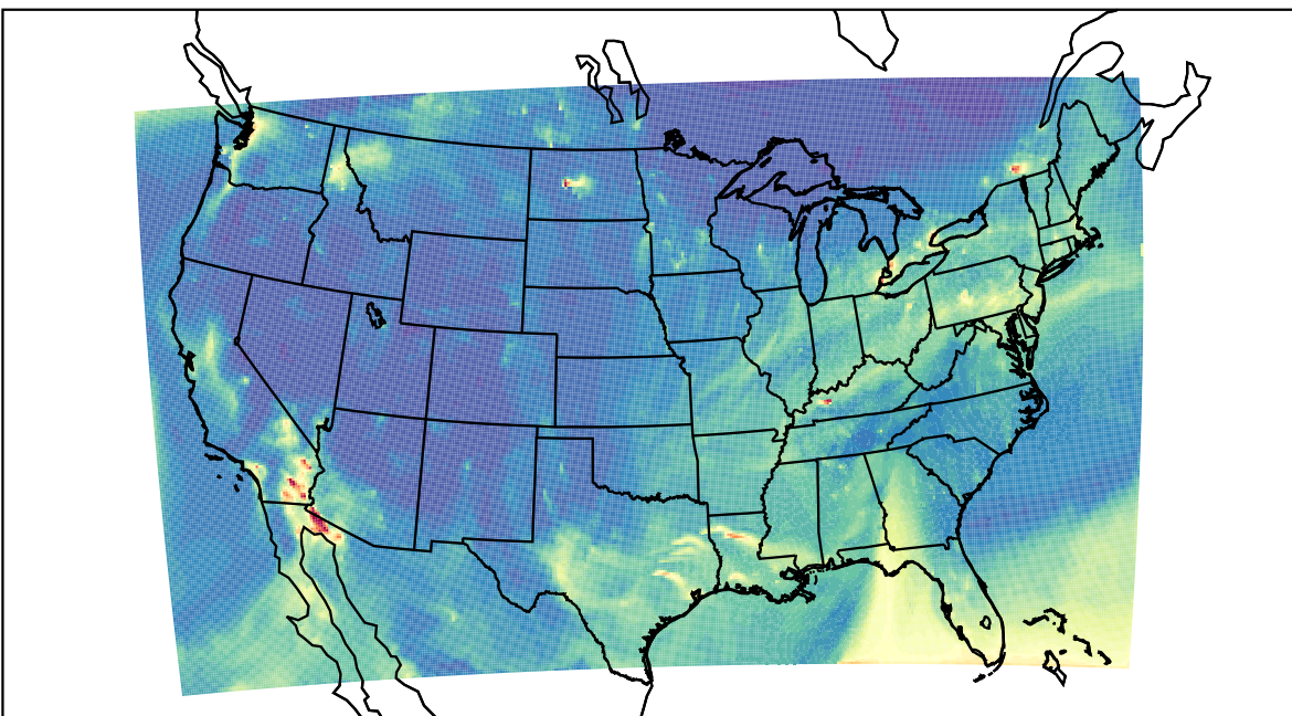
WRF 2020-10-29_12:00:00
