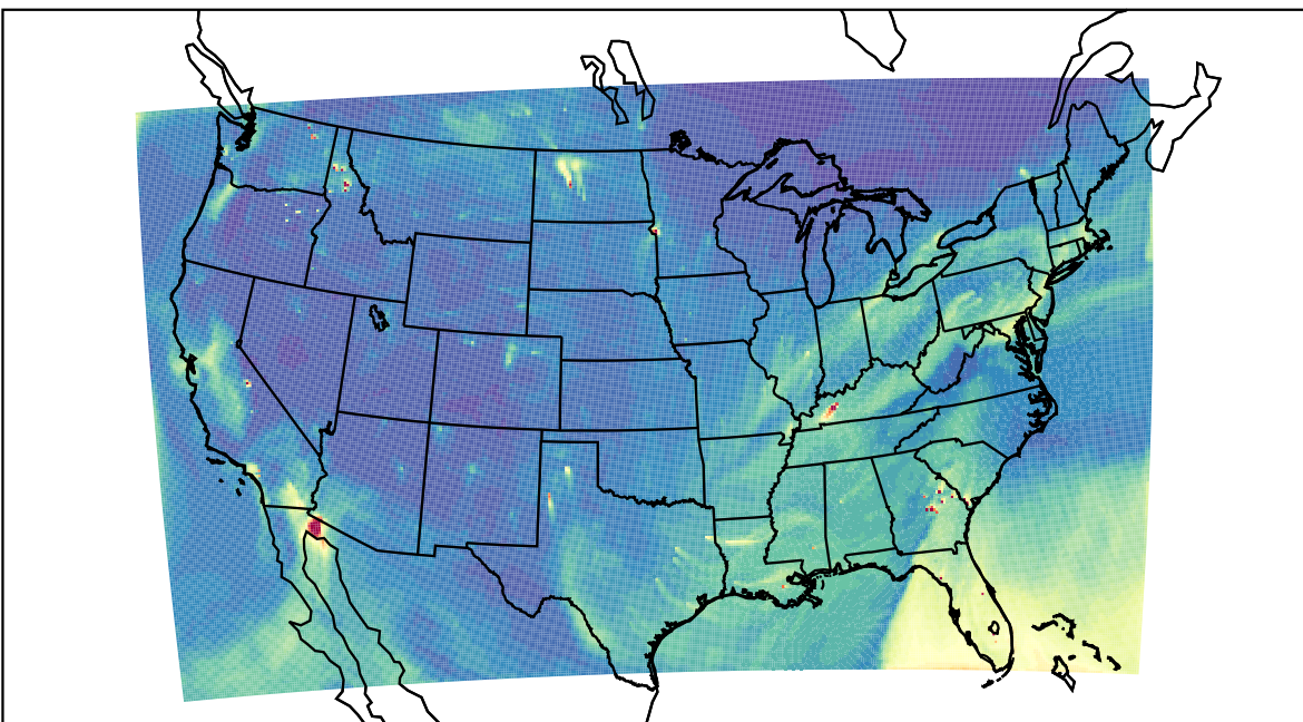
WRF 2020-10-29_19:00:00
