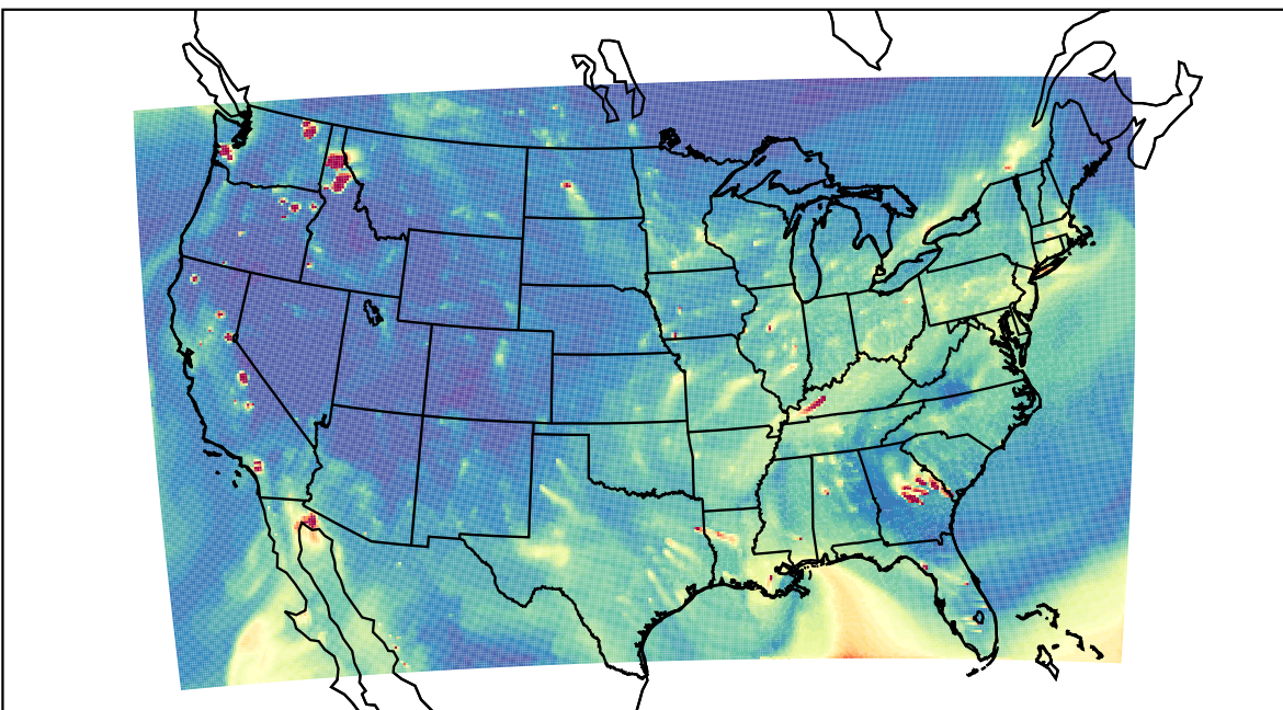
WRF 2020-10-29_00:00:00
