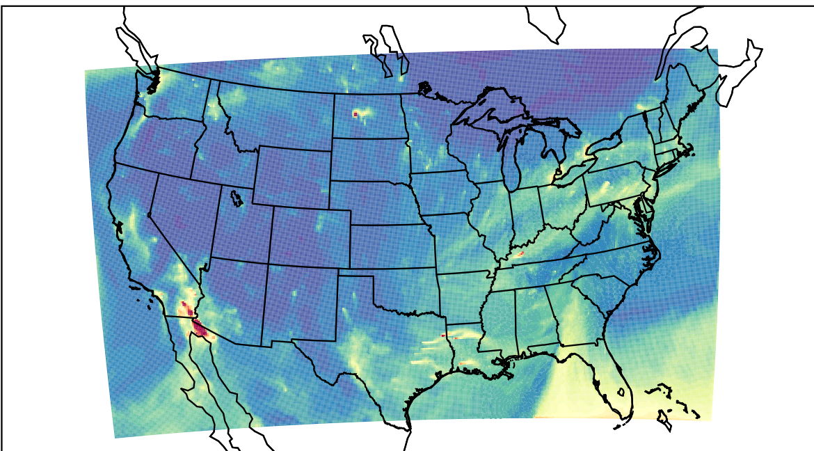
WRF 2020-10-29_14:00:00
