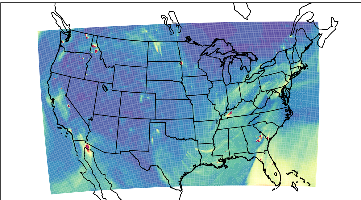
WRF 2020-10-29_21:00:00
