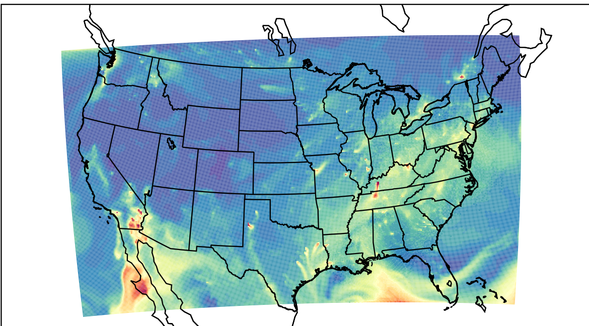
WRF 2020-10-28_12:00:00
