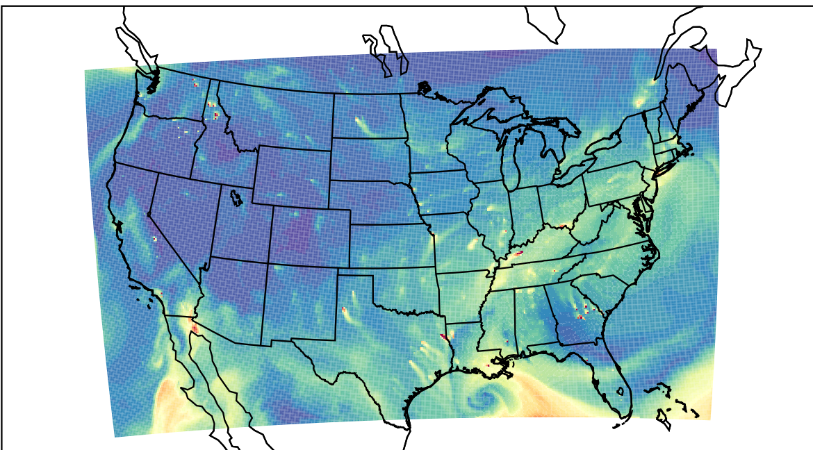
WRF 2020-10-28_19:00:00
