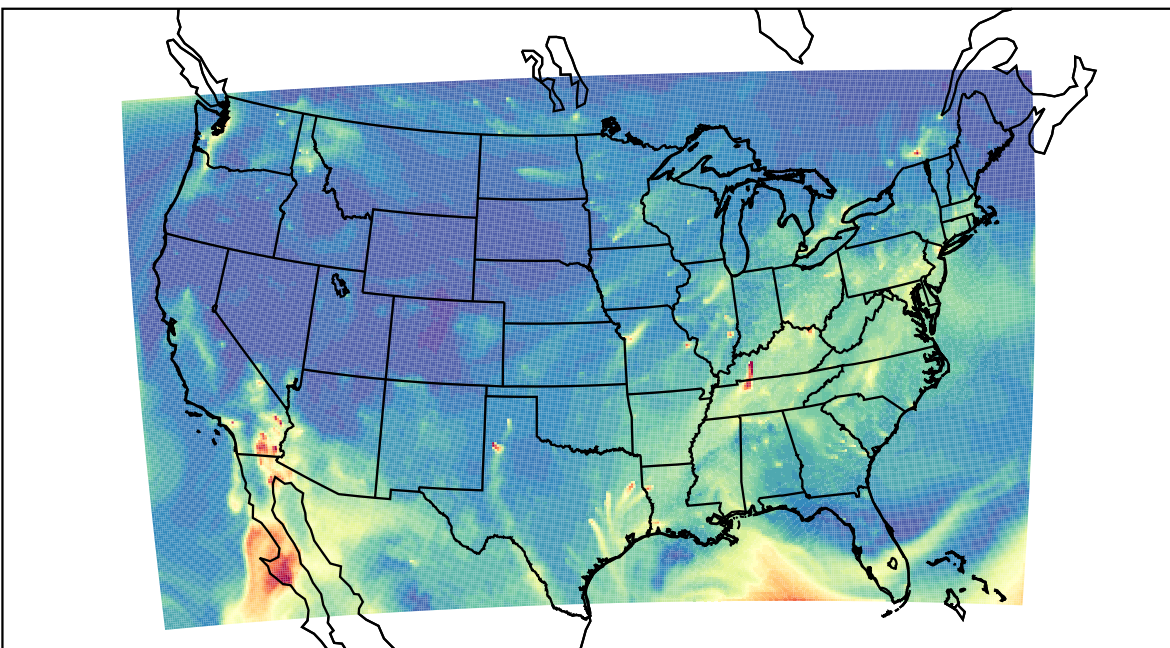
WRF 2020-10-28_11:00:00
