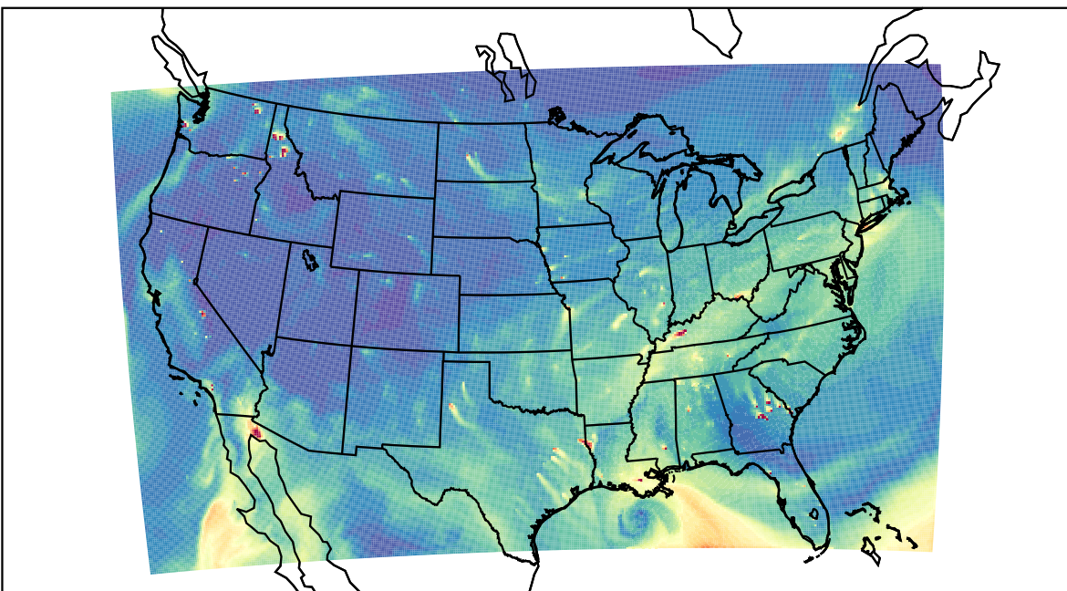
WRF 2020-10-28_20:00:00
