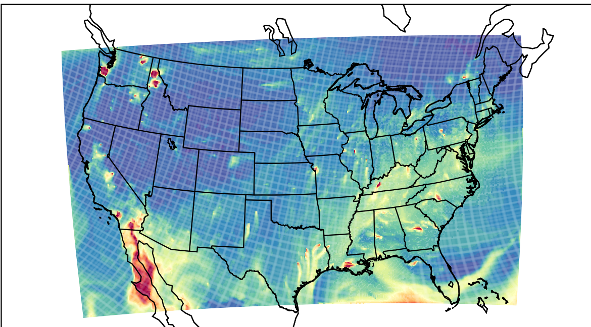
WRF 2020-10-28_04:00:00
