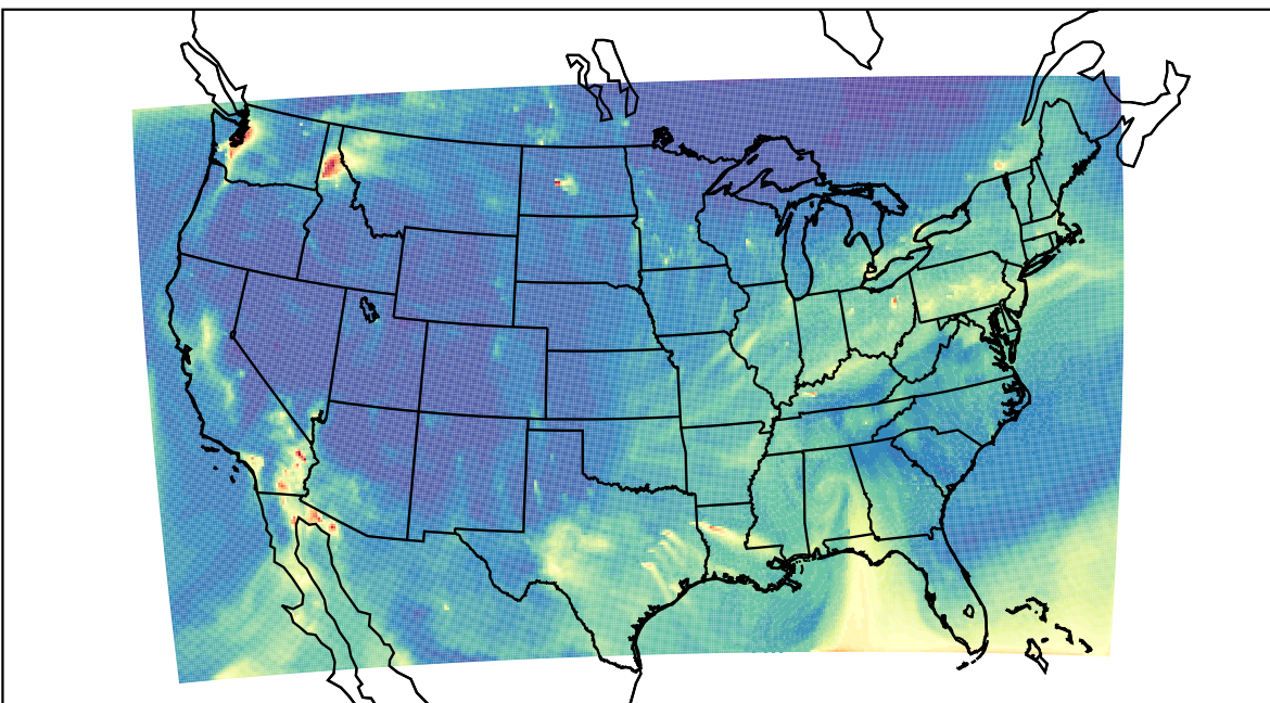
WRF 2020-10-29_09:00:00
