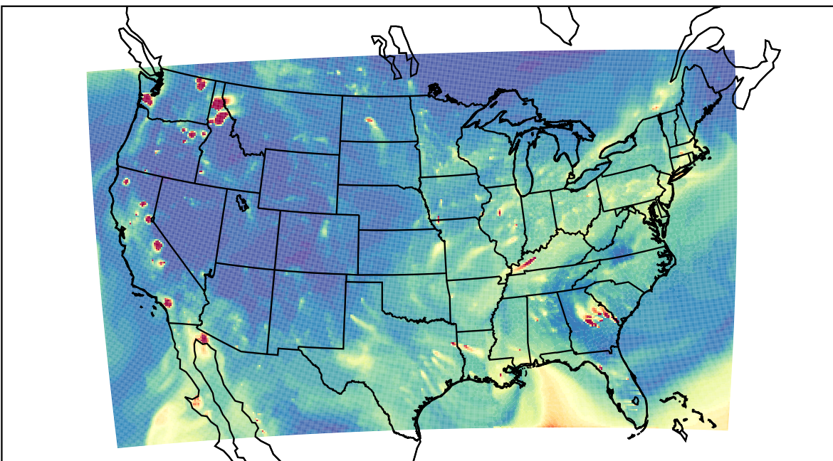
WRF 2020-10-29_01:00:00
