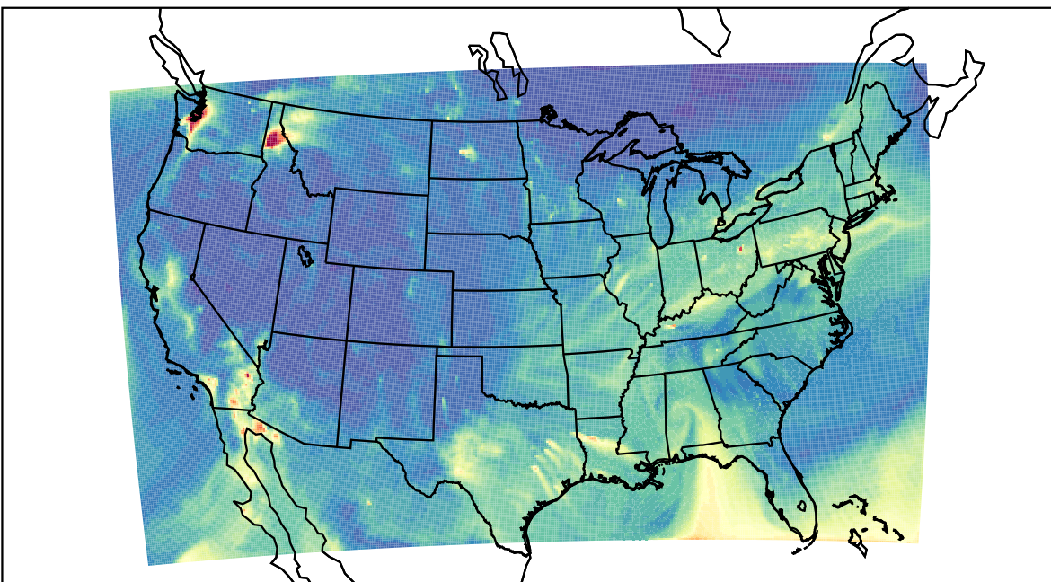
WRF 2020-10-29_08:00:00
