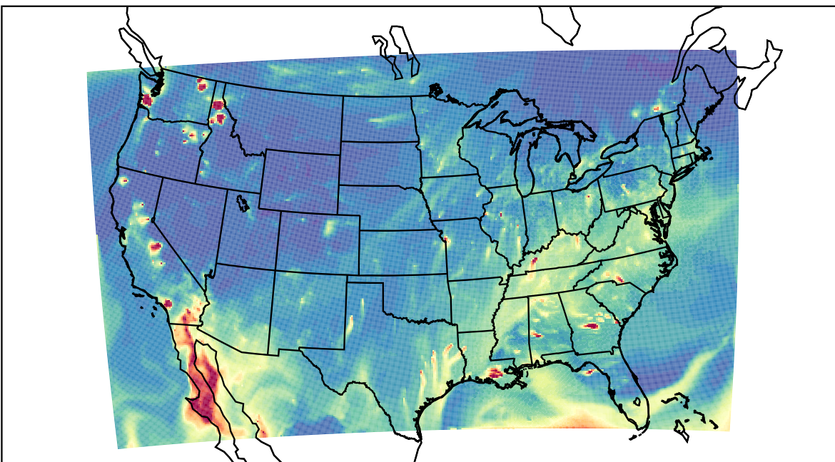
WRF 2020-10-28_03:00:00
