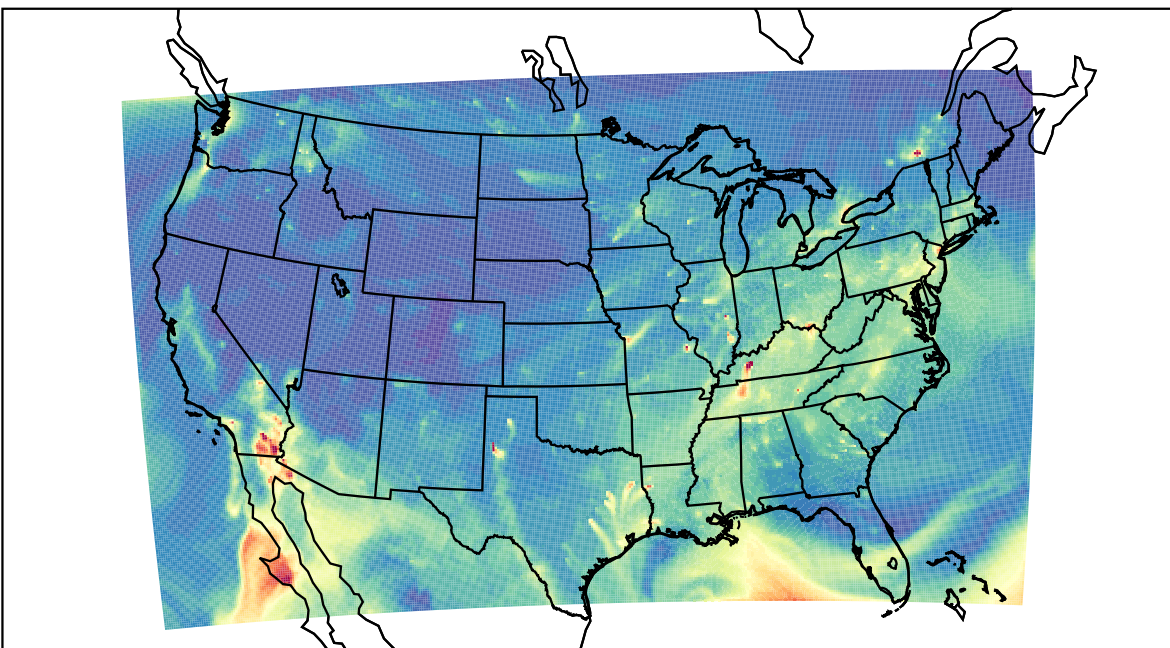
WRF 2020-10-28_13:00:00
