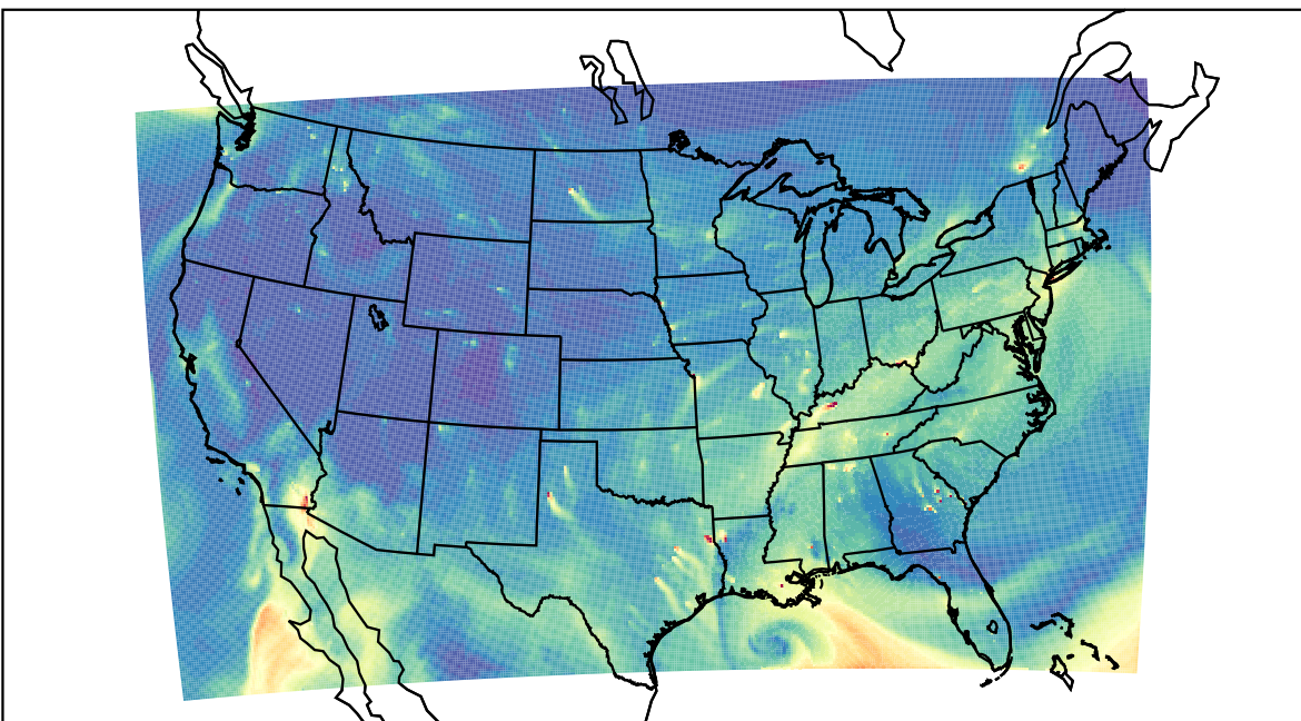
WRF 2020-10-28_18:00:00
