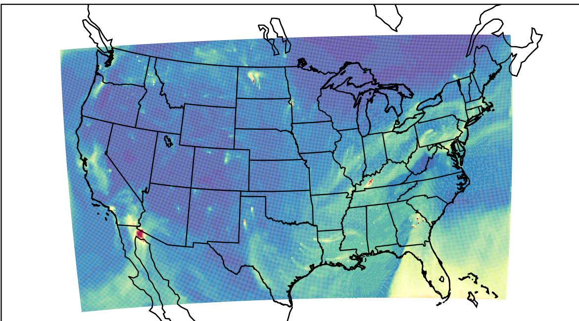
WRF 2020-10-29_18:00:00
