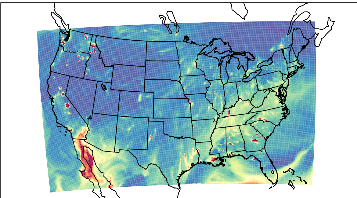
WRF 2020-10-28_01:00:00
