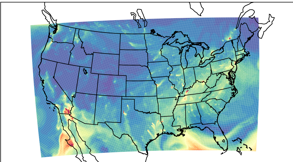
WRF 2020-10-28_14:00:00
