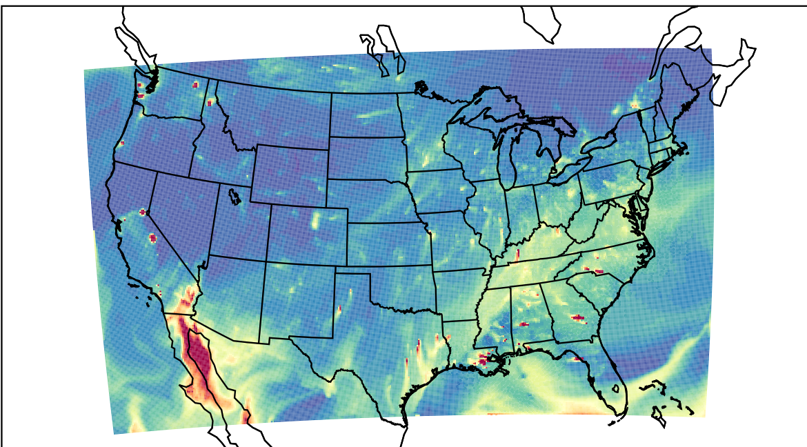
WRF 2020-10-28_00:00:00
