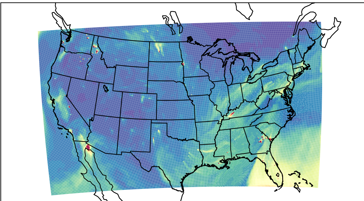
WRF 2020-10-29_20:00:00
