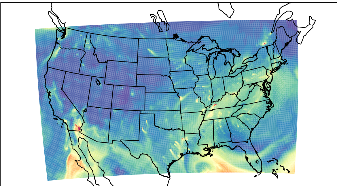
WRF 2020-10-28_16:00:00
