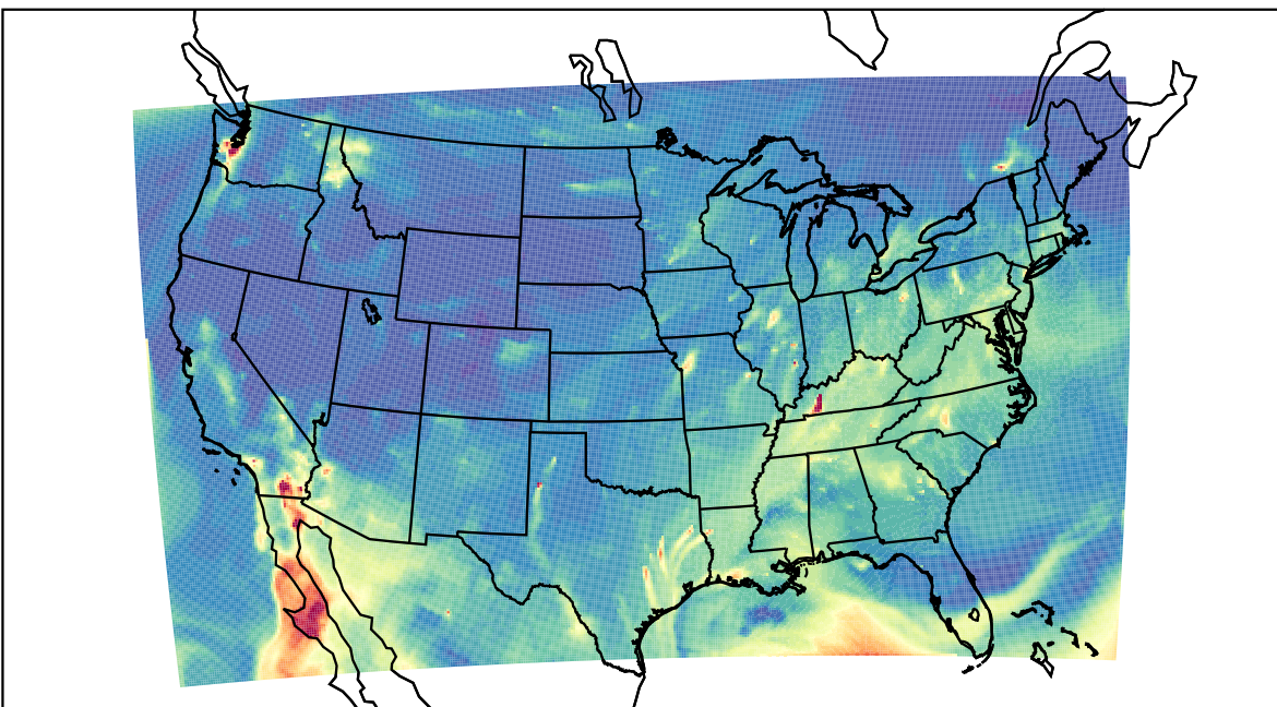
WRF 2020-10-28_08:00:00
