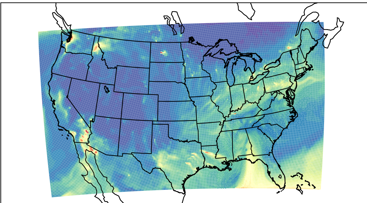
WRF 2020-10-29_10:00:00
