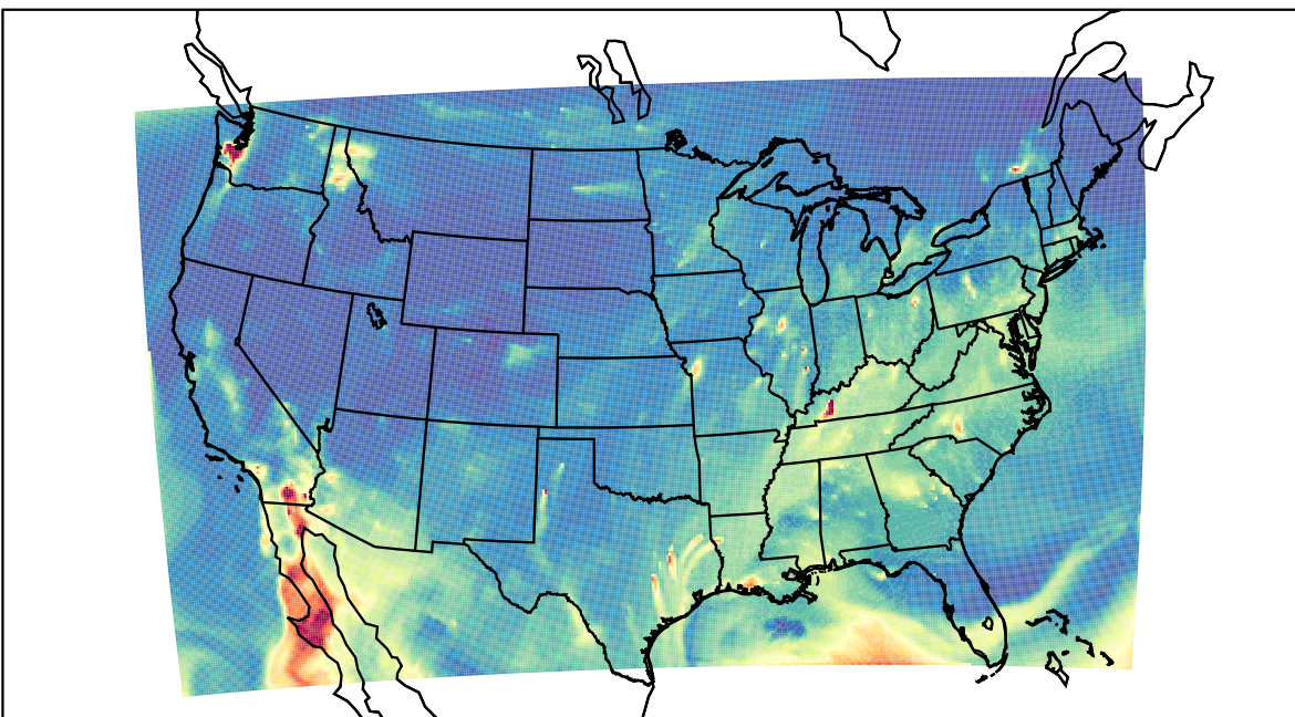
WRF 2020-10-28_07:00:00
