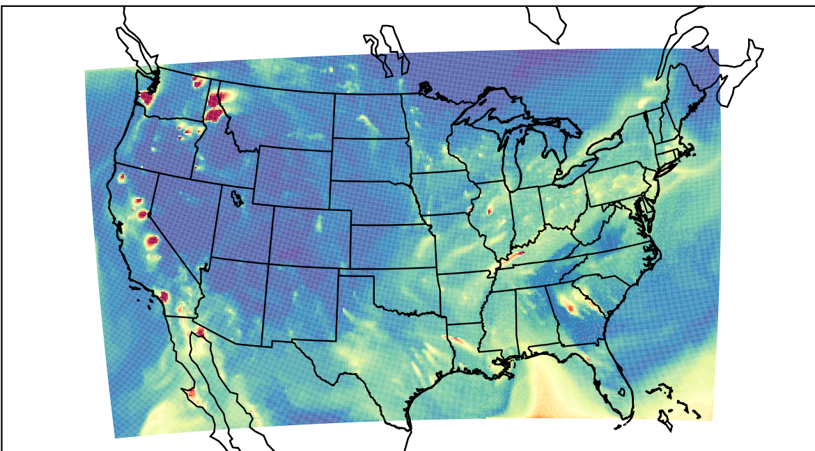
WRF 2020-10-29_03:00:00
