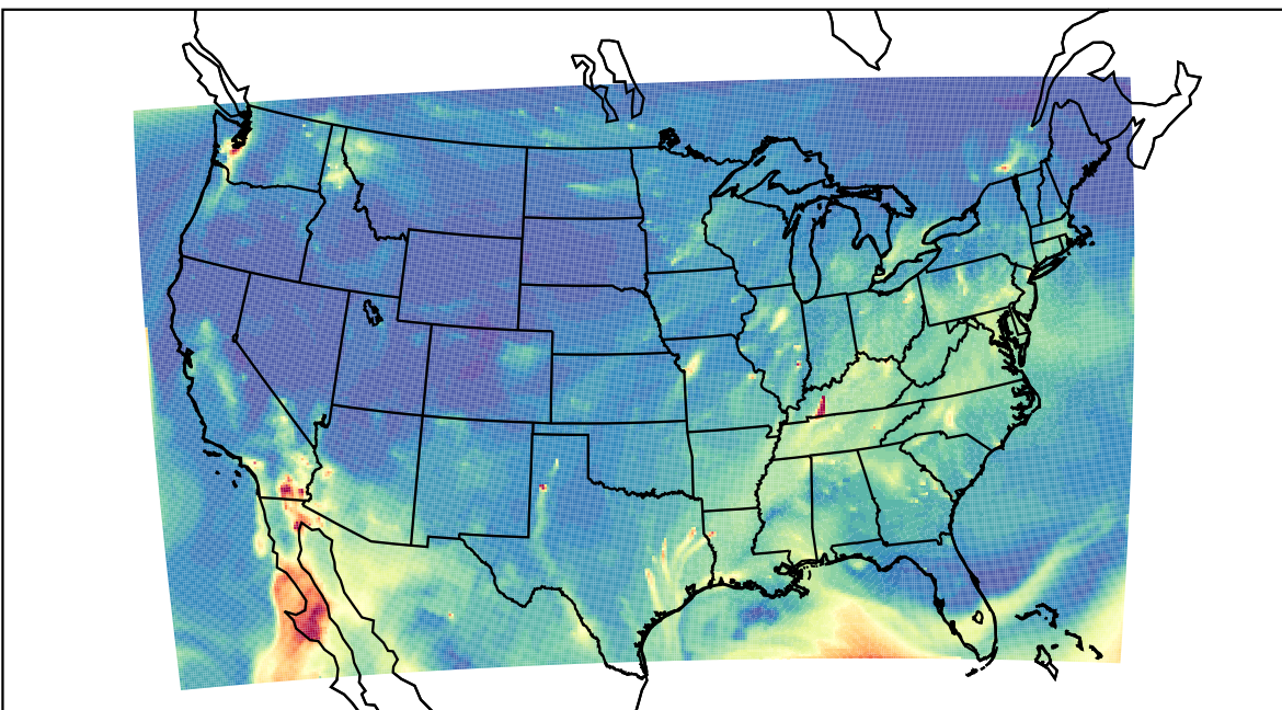
WRF 2020-10-28_09:00:00
