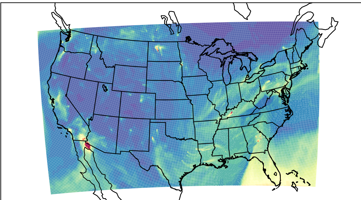
WRF 2020-10-29_17:00:00
