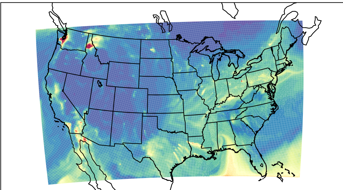
WRF 2020-10-29_07:00:00
