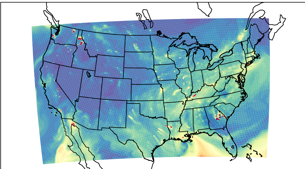
WRF 2020-10-28_22:00:00
