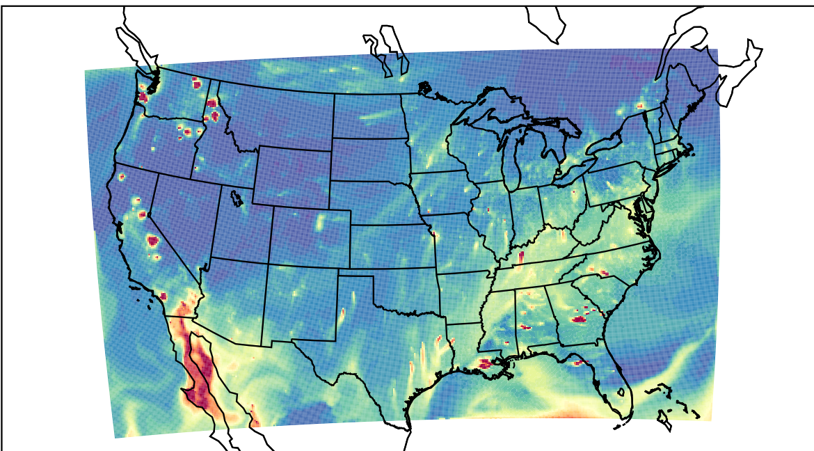
WRF 2020-10-28_02:00:00
