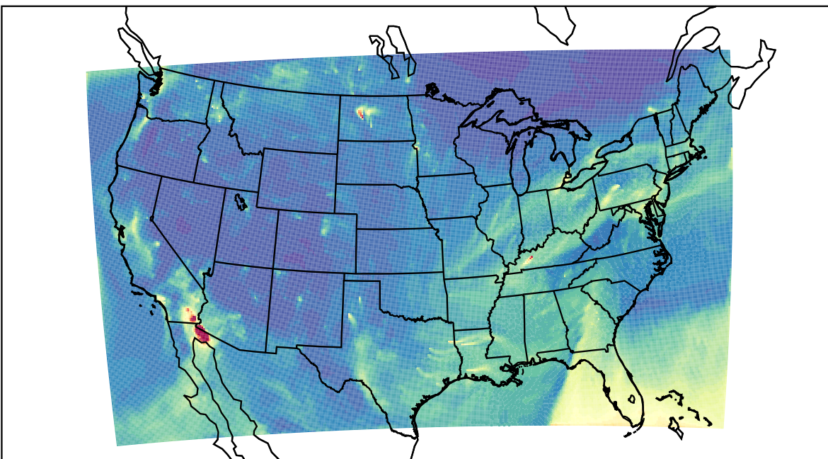
WRF 2020-10-29_16:00:00
