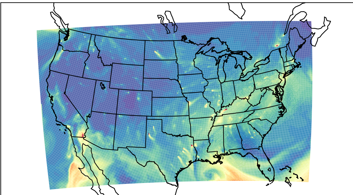
WRF 2020-10-28_17:00:00
