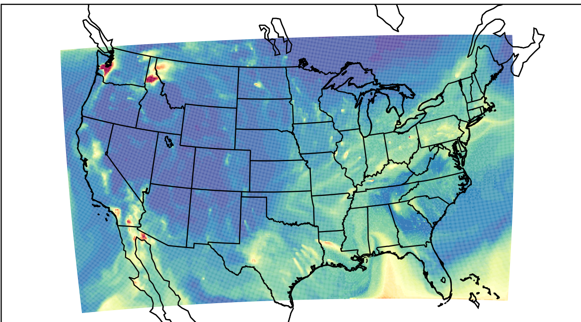
WRF 2020-10-29_06:00:00
