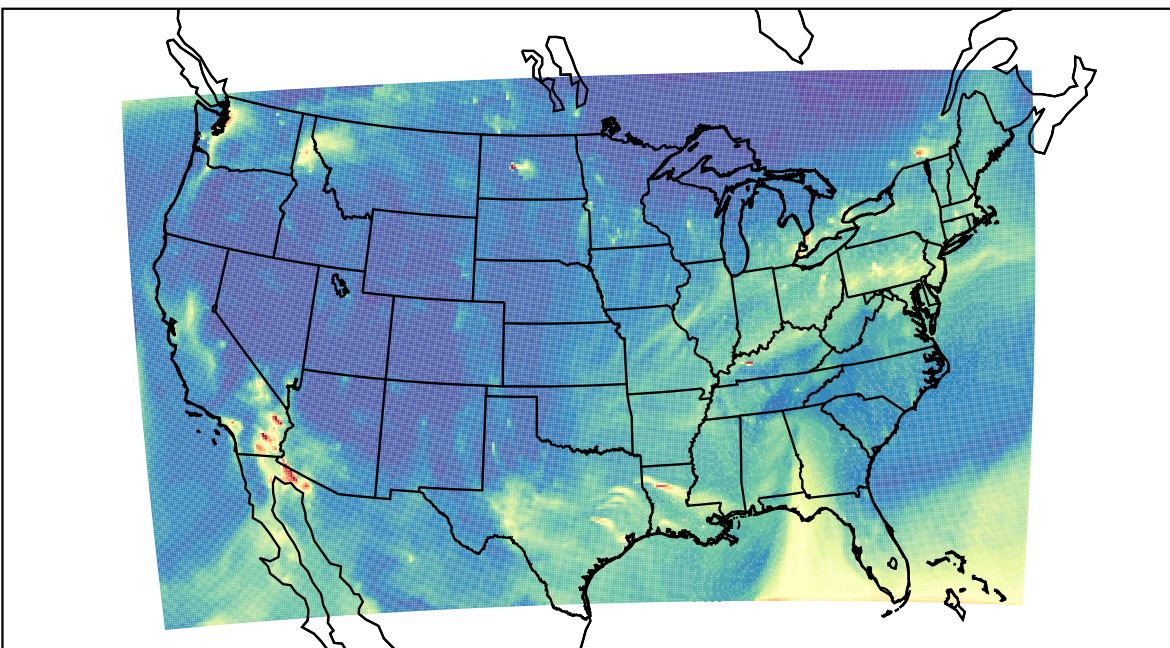
WRF 2020-10-29_11:00:00
