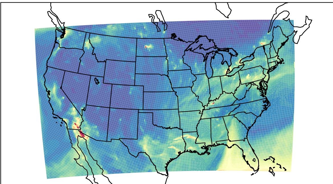
WRF 2020-10-29_13:00:00
