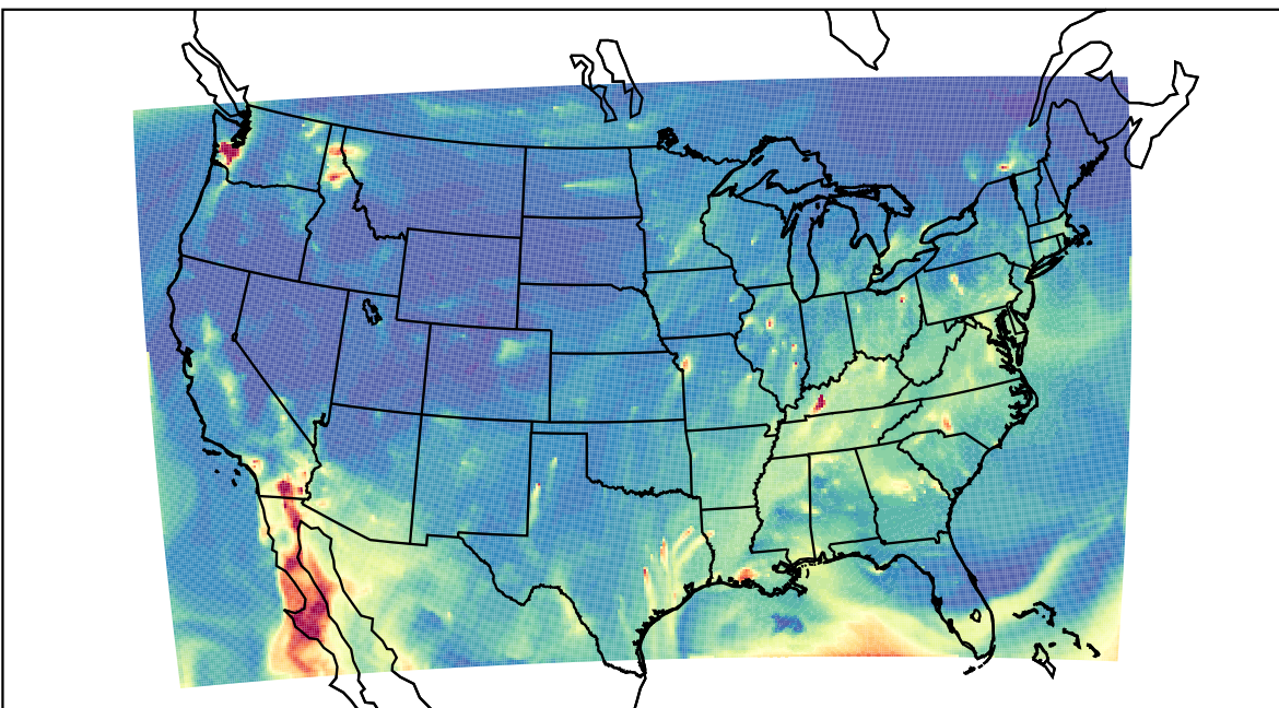
WRF 2020-10-28_06:00:00
