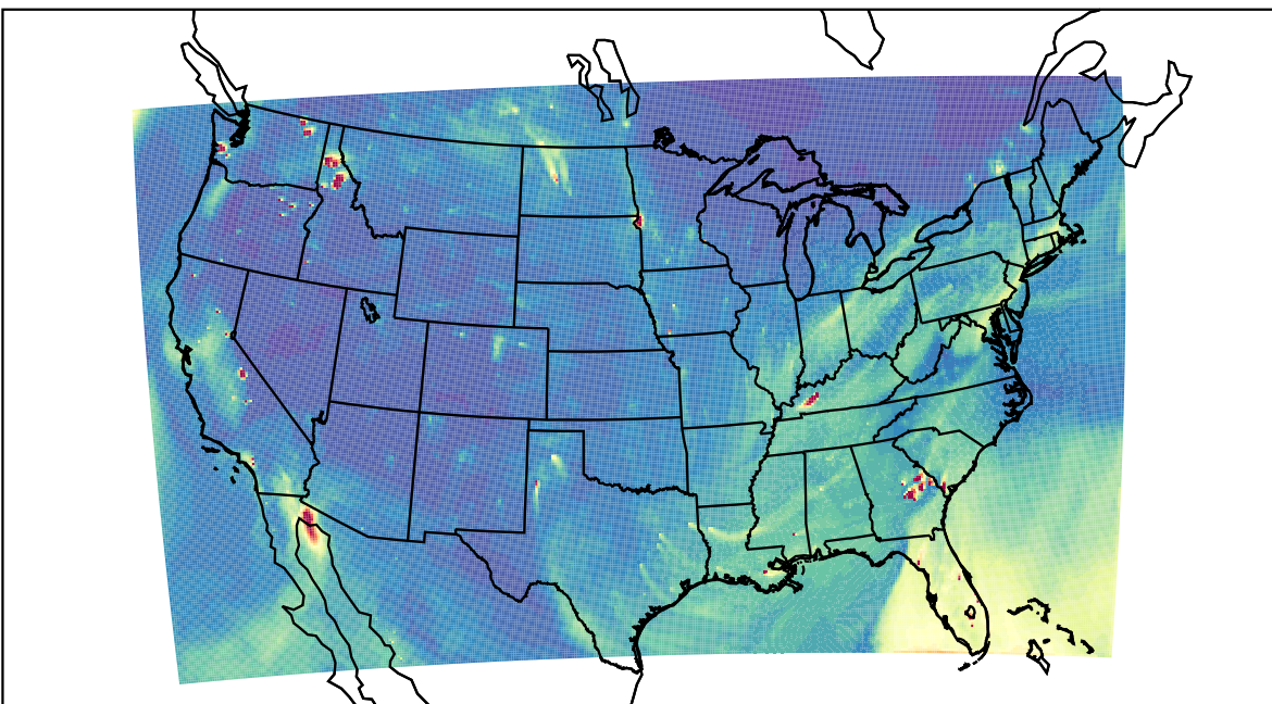
WRF 2020-10-29_22:00:00
