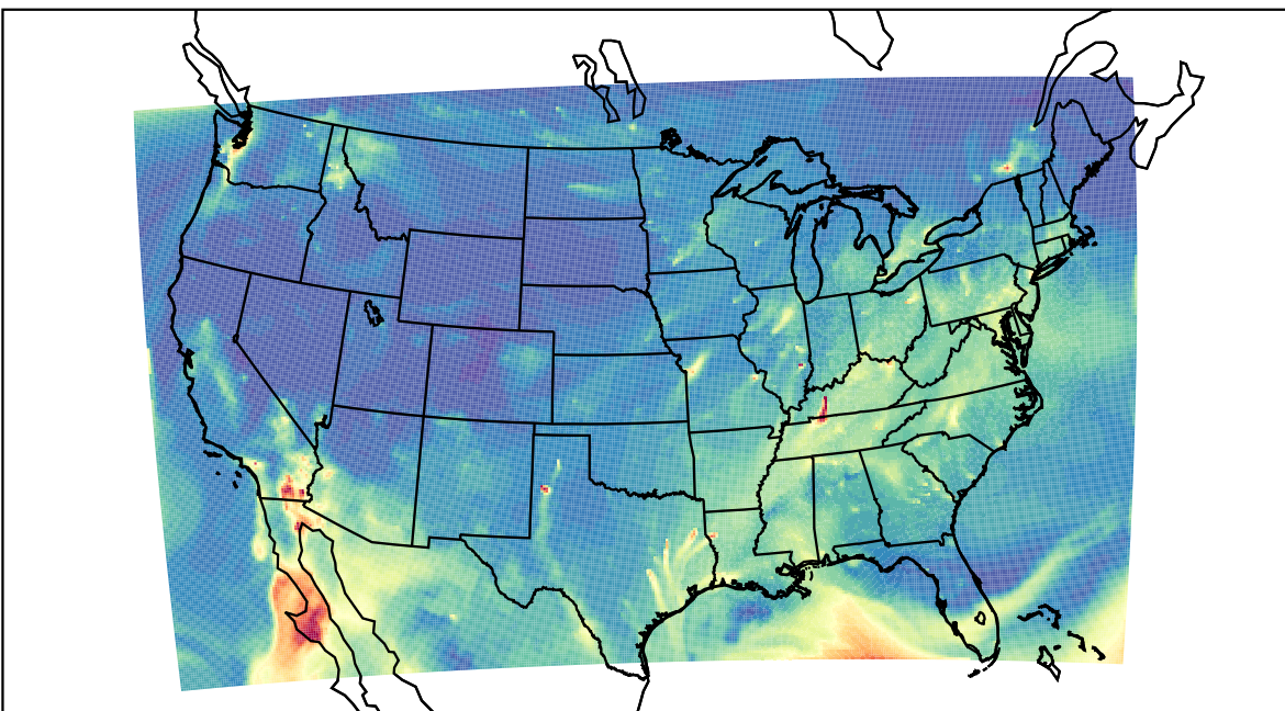
WRF 2020-10-28_10:00:00
