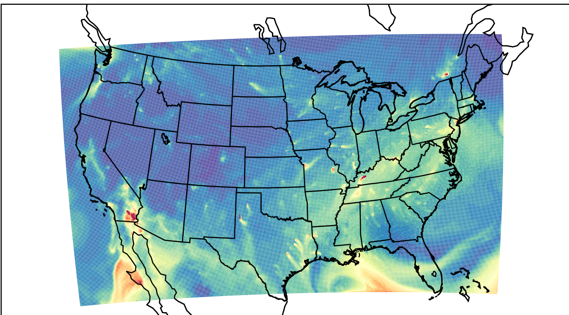
WRF 2020-10-28_15:00:00
