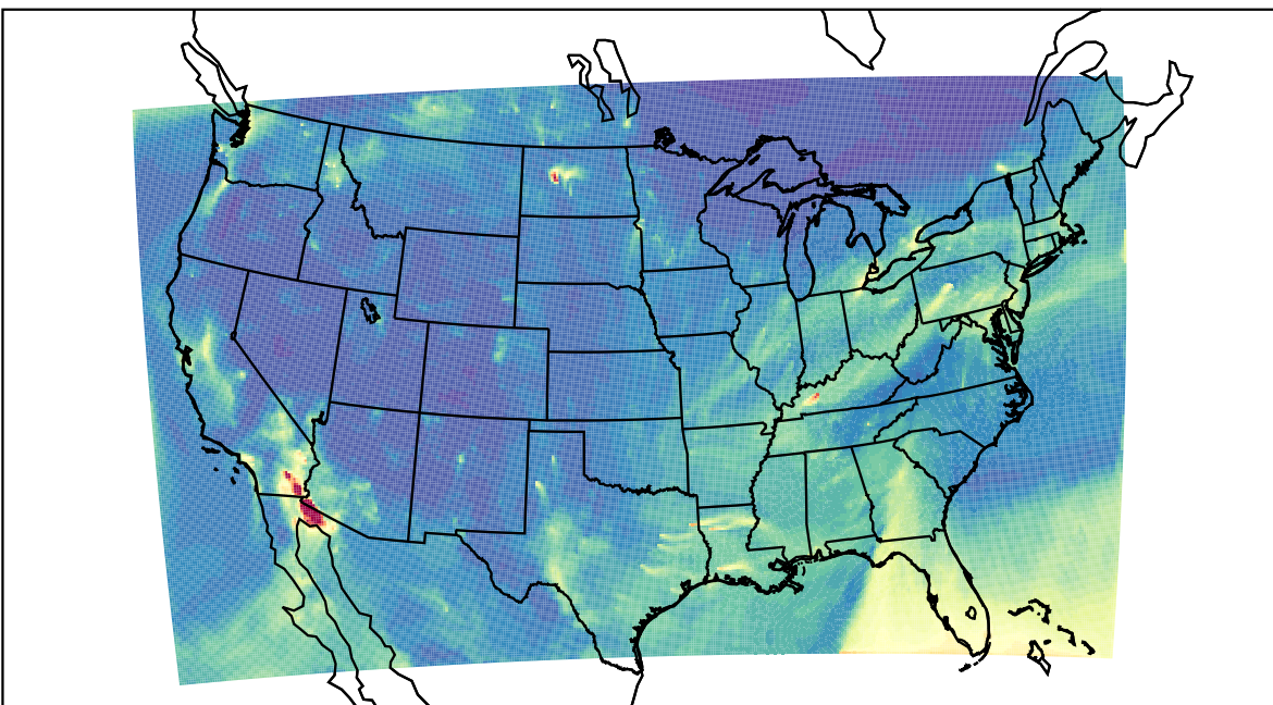
WRF 2020-10-29_15:00:00
