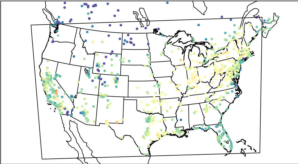
AirNOW (2020-11-06_18:00:00)
