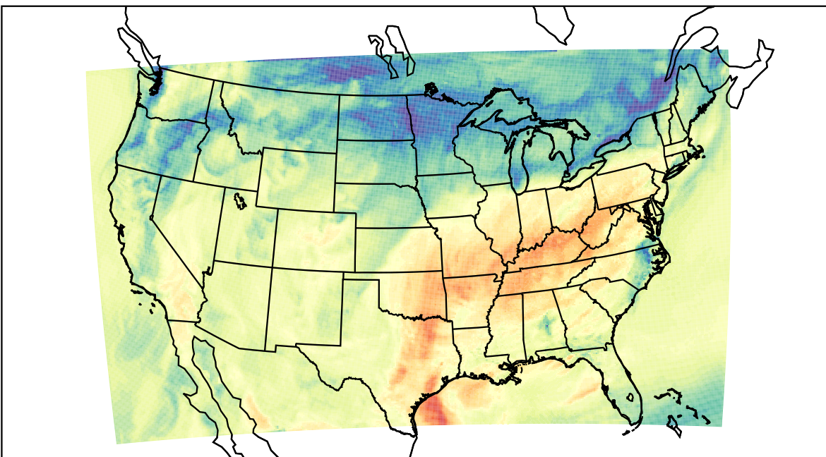
WRF (2020-11-06_20:00:00)
