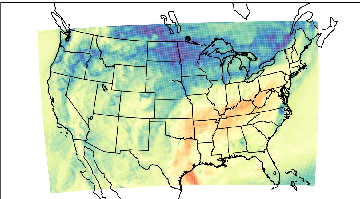
WRF (2020-11-06_18:00:00)
