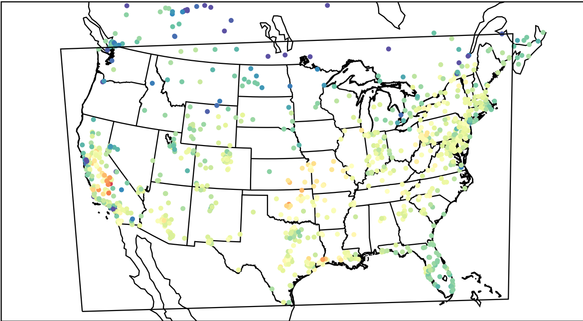
AirNOW (2020-11-05_20:00:00)
