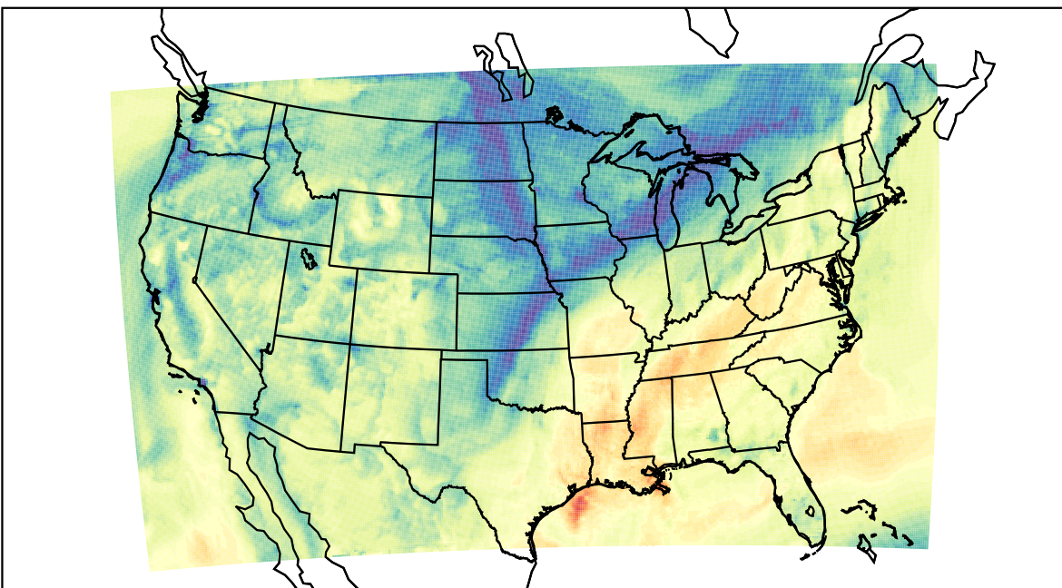
WRF (2020-11-05_18:00:00)
