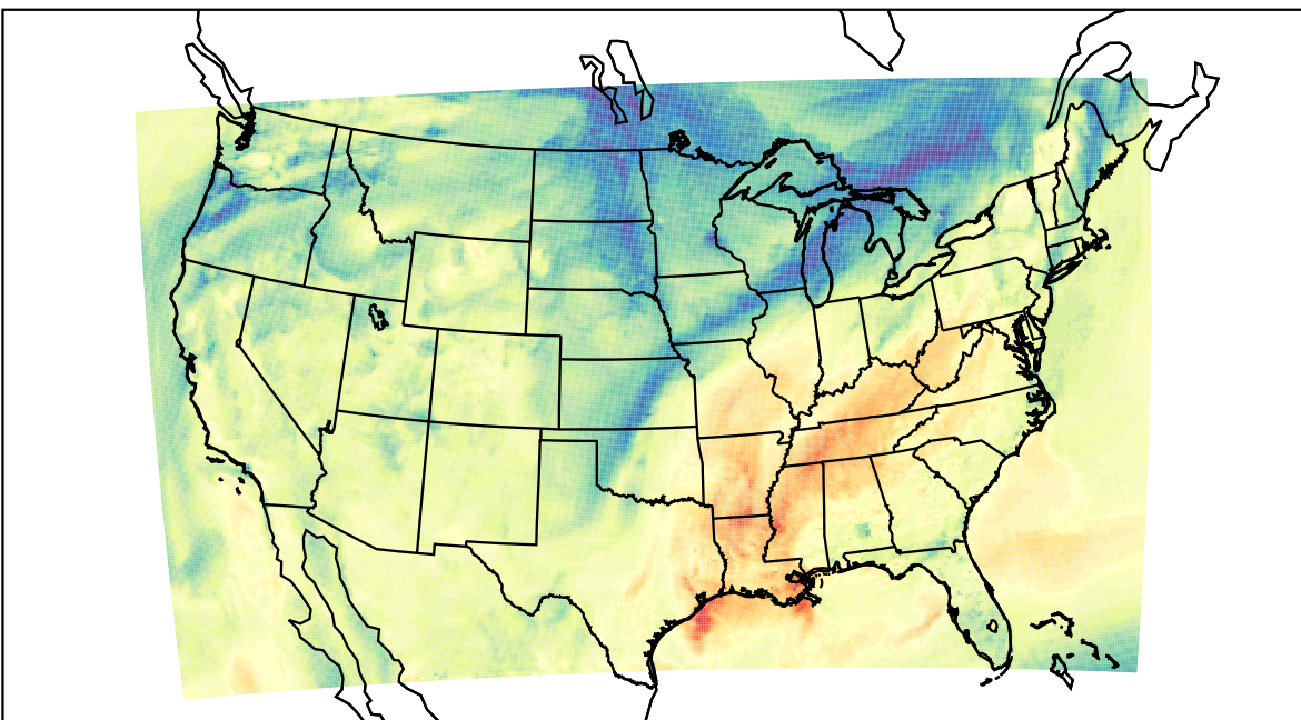
WRF (2020-11-05_20:00:00)
