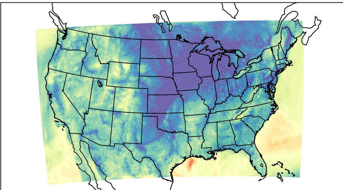
WRF (2020-11-05_13:00:00)
