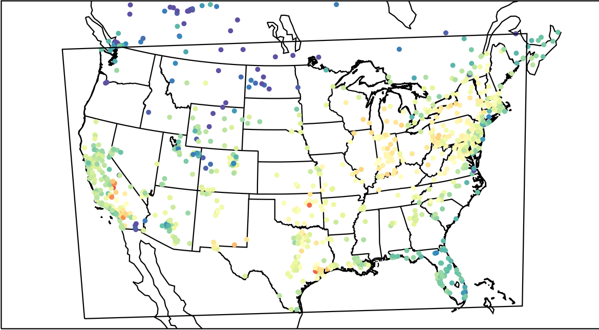
AirNOW (2020-11-06_20:00:00)
