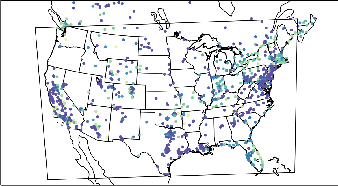
AirNOW (2020-11-05_13:00:00)
