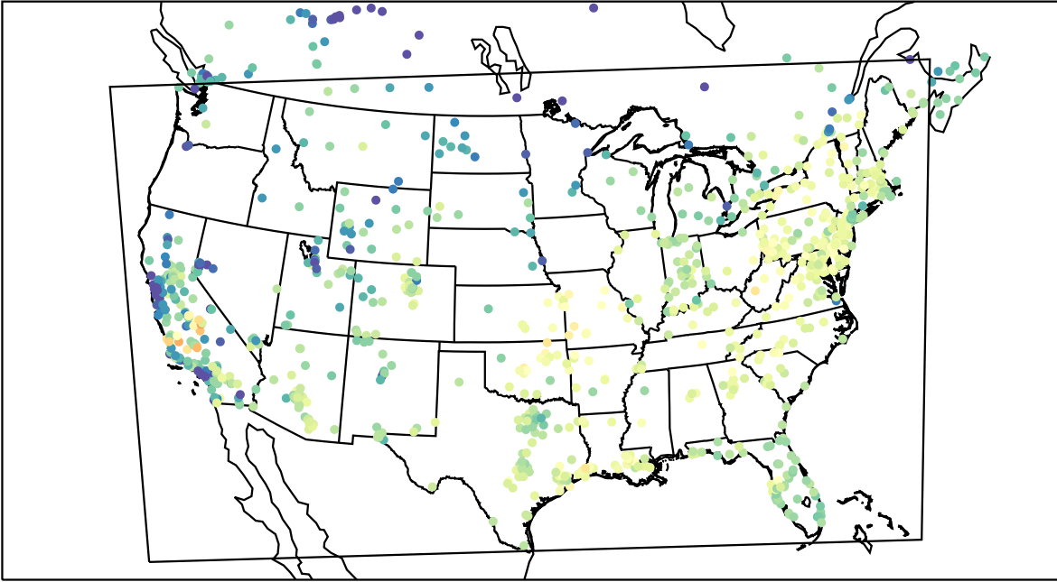
AirNOW (2020-11-05_18:00:00)
