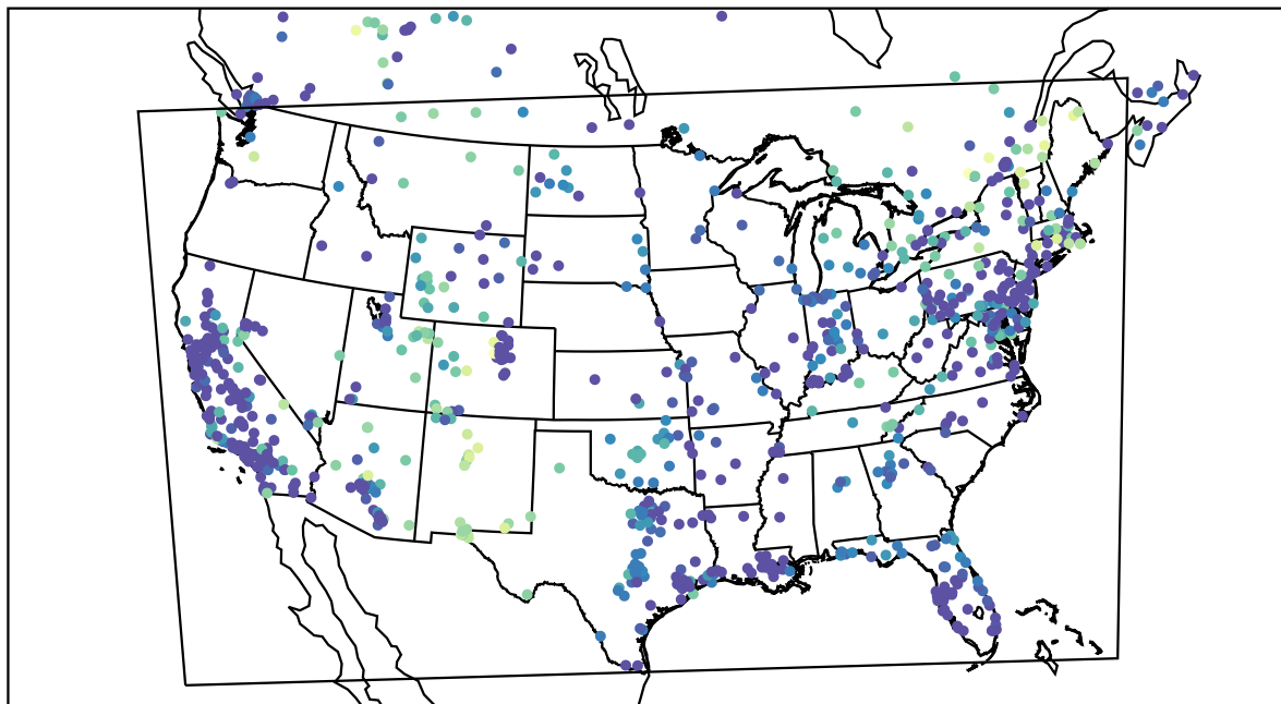
AirNOW (2020-11-10_04:00:00)
