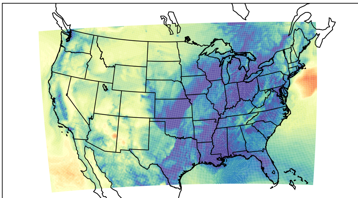
WRF (2020-11-10_13:00:00)
