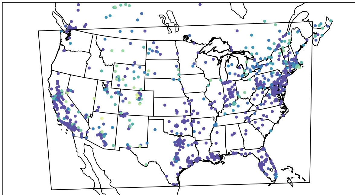
AirNOW (2020-11-11_10:00:00)
