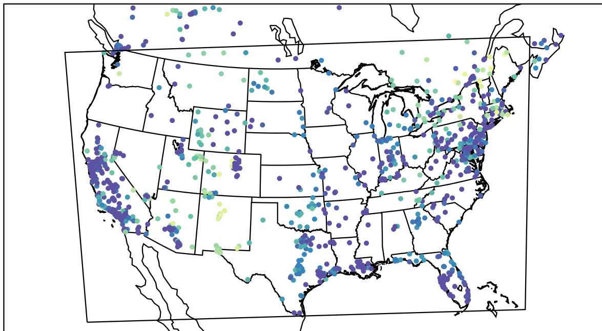
AirNOW (2020-11-10_03:00:00)
