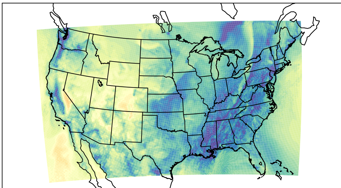
WRF (2020-11-11_16:00:00)
