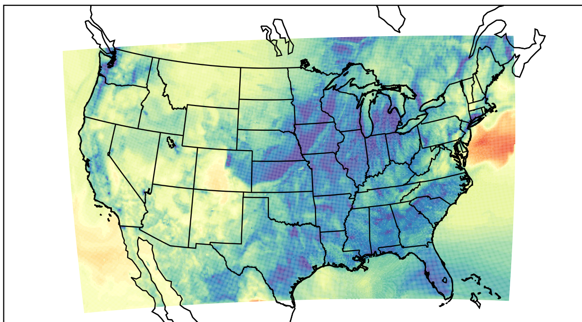
WRF (2020-11-10_03:00:00)
