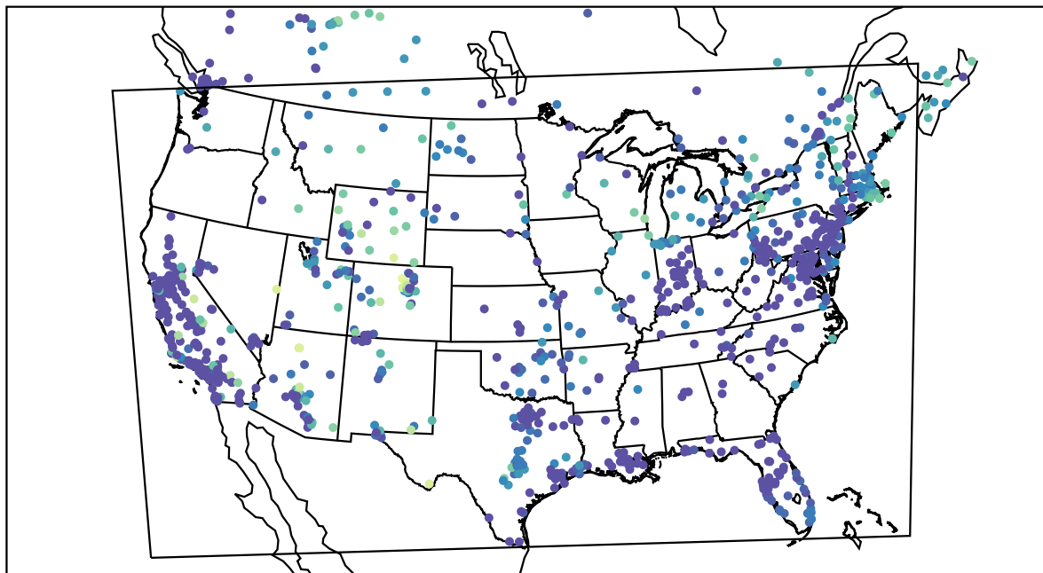
AirNOW (2020-11-11_15:00:00)
