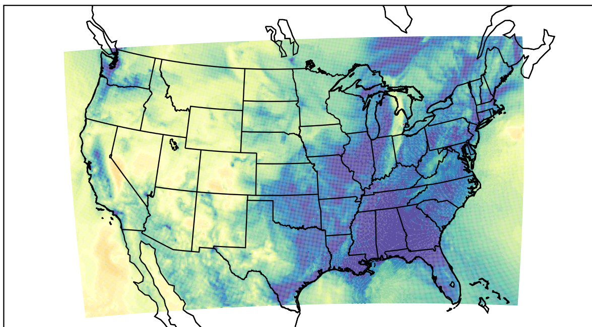
WRF (2020-11-11_08:00:00)
