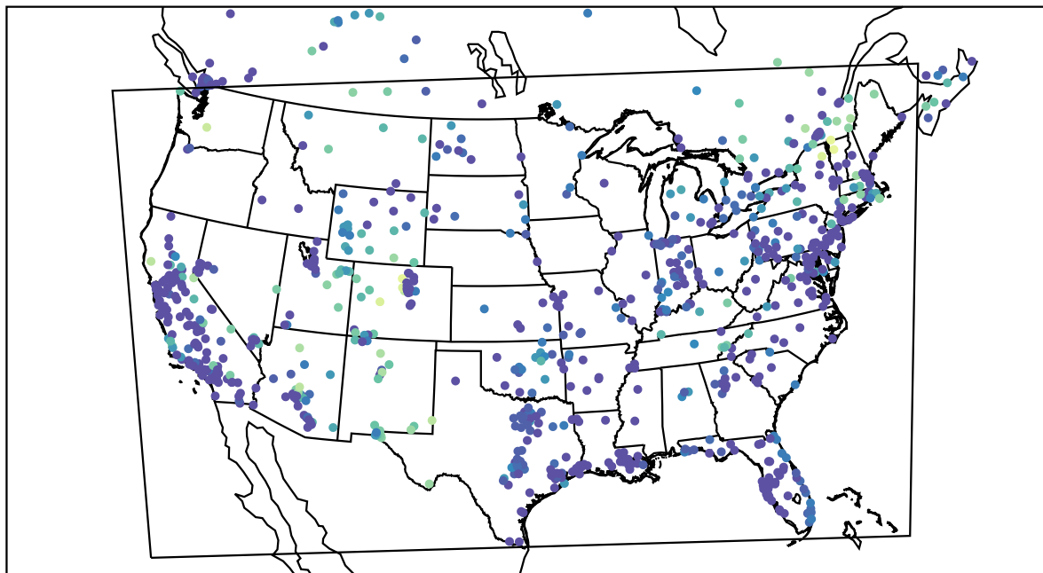
AirNOW (2020-11-10_10:00:00)
