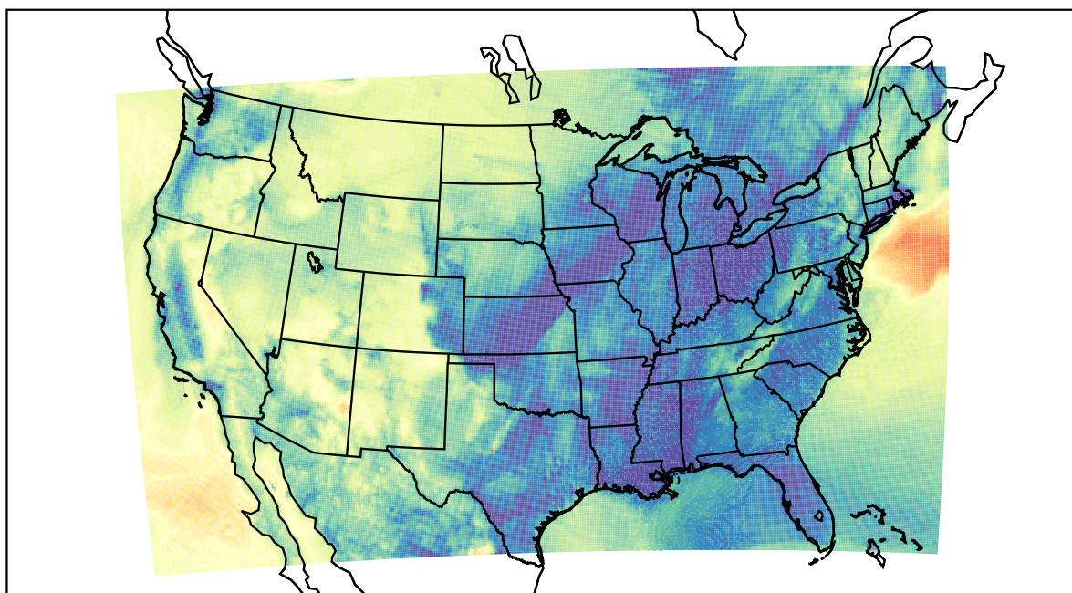
WRF (2020-11-10_10:00:00)
