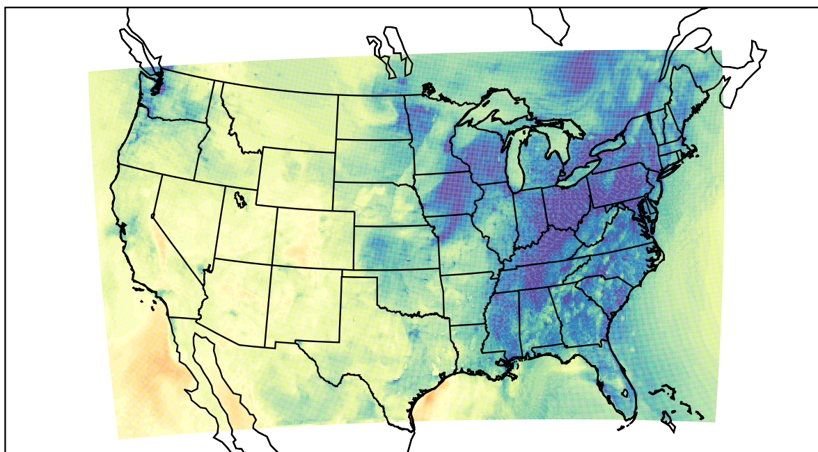
WRF (2020-11-11_23:00:00)
