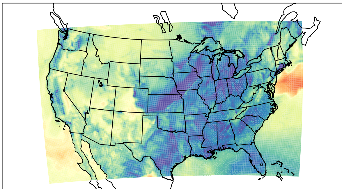
WRF (2020-11-10_06:00:00)
