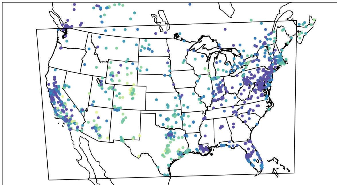
AirNOW (2020-11-11_17:00:00)
