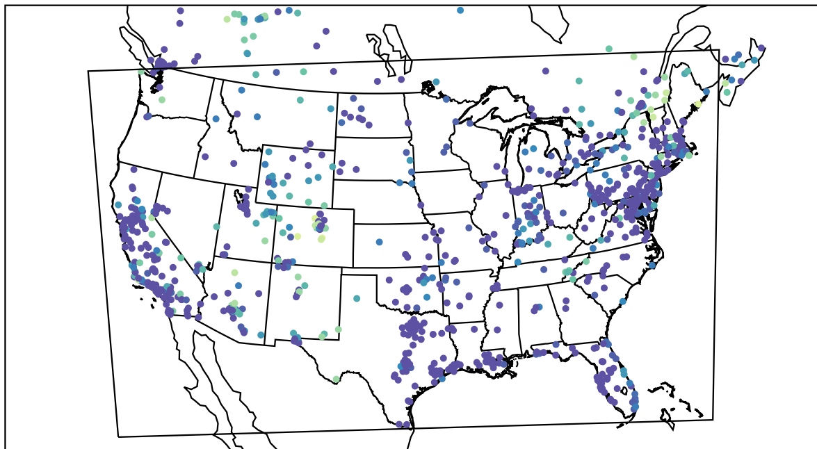
AirNOW (2020-11-10_13:00:00)
