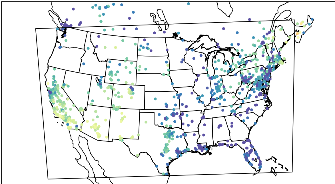
AirNOW (2020-11-10_23:00:00)
