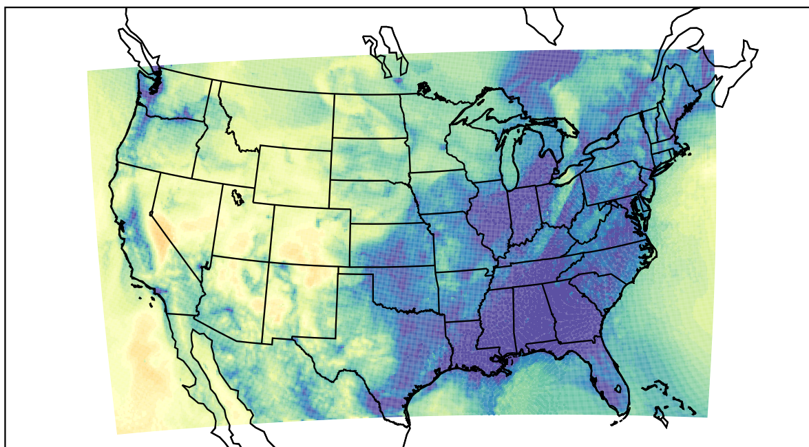
WRF (2020-11-11_12:00:00)
