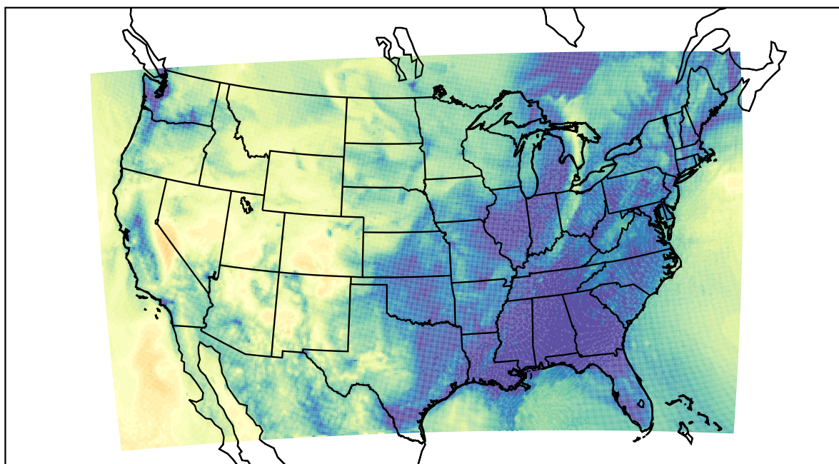
WRF (2020-11-11_10:00:00)
