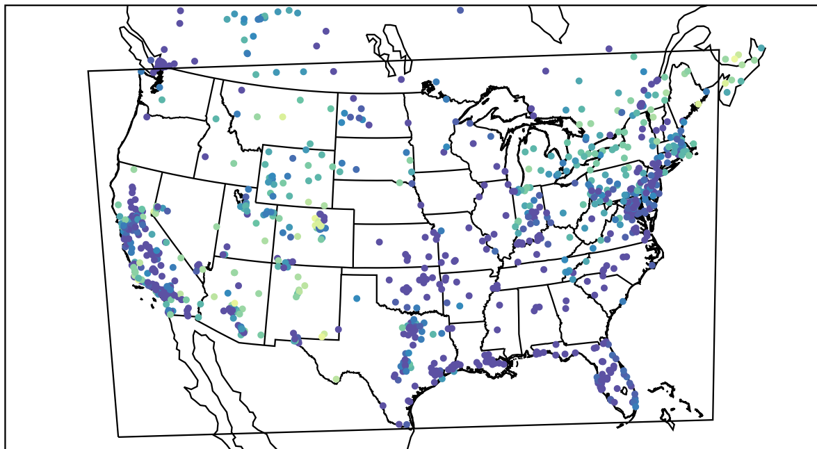
AirNOW (2020-11-11_03:00:00)
