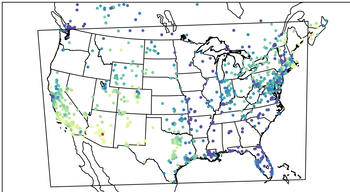
AirNOW (2020-11-10_22:00:00)
