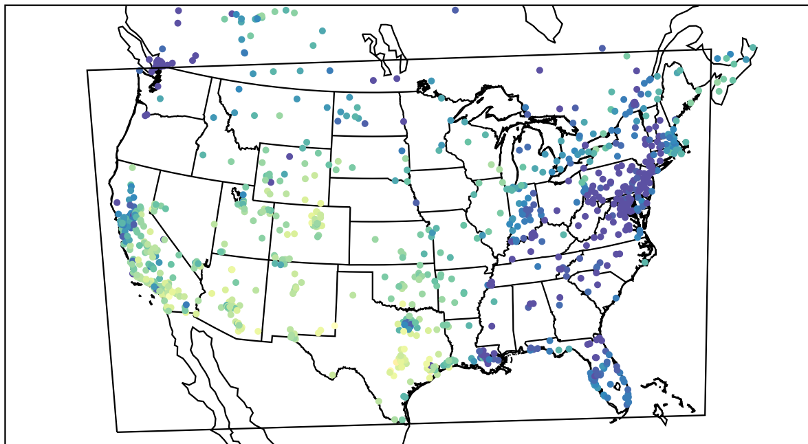
AirNOW (2020-11-11_19:00:00)
