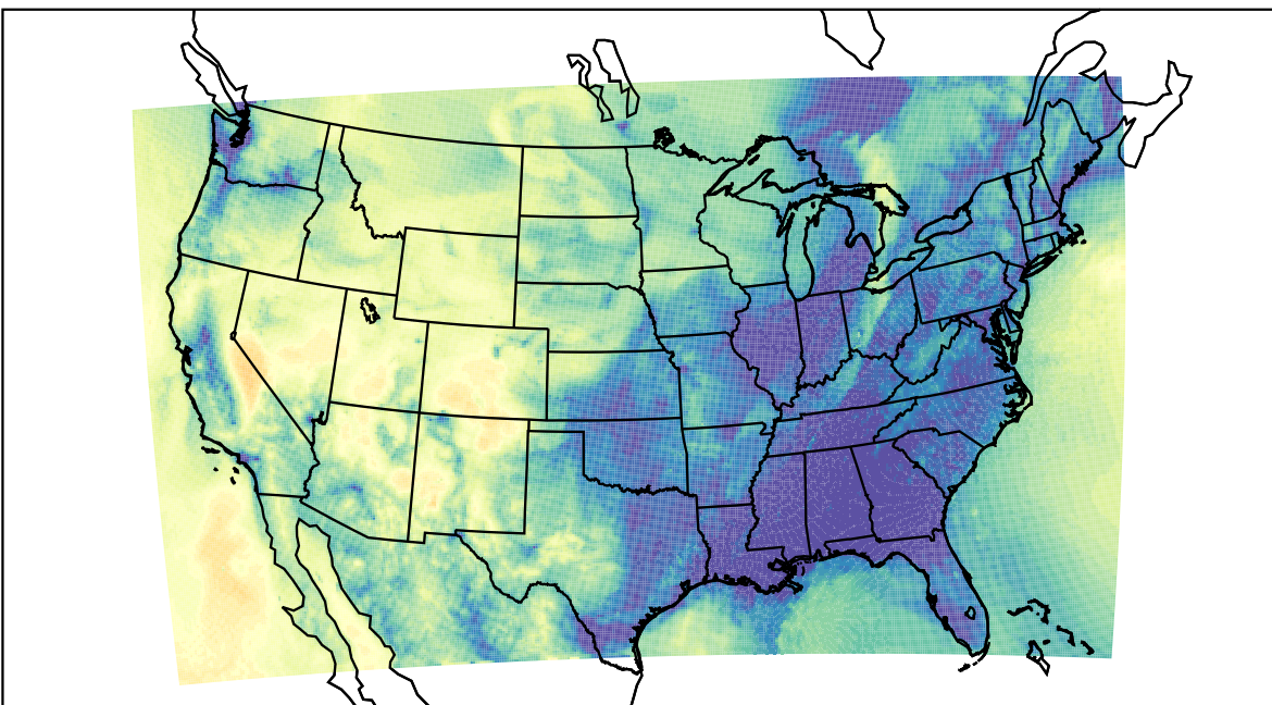
WRF (2020-11-11_11:00:00)
