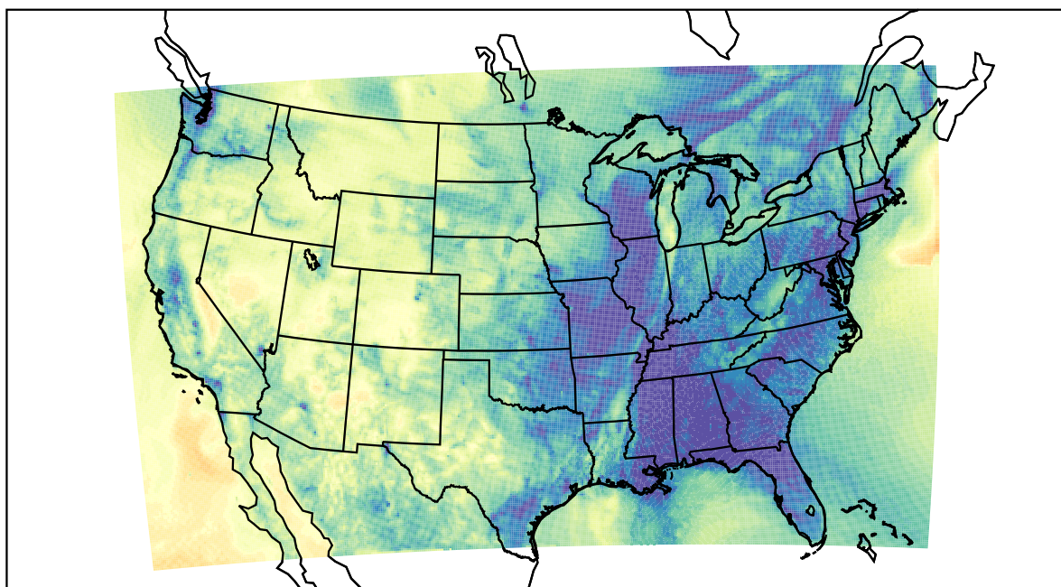
WRF (2020-11-11_03:00:00)
