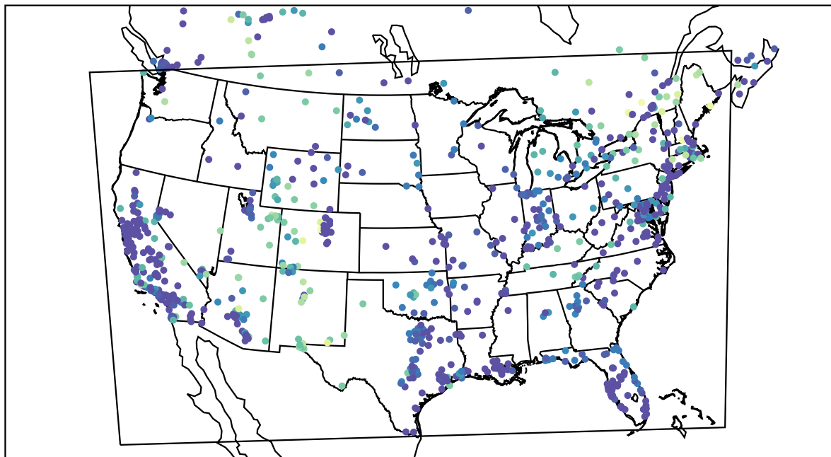
AirNOW (2020-11-10_06:00:00)
