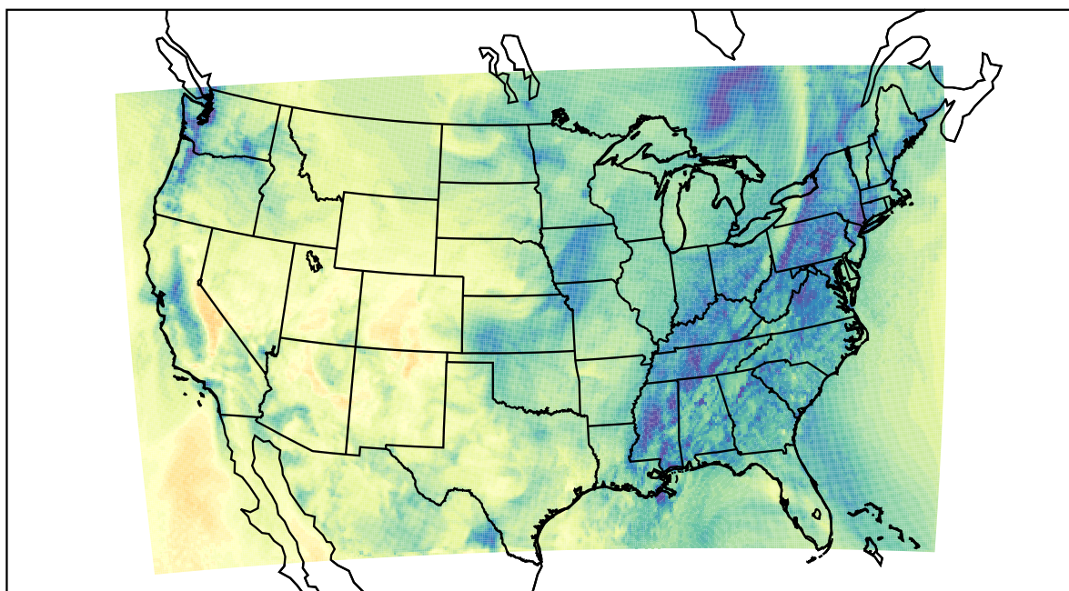
WRF (2020-11-11_18:00:00)
