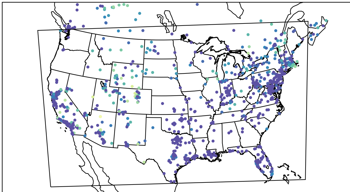
AirNOW (2020-11-11_12:00:00)
