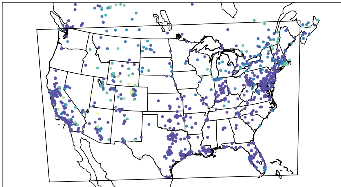
AirNOW (2020-11-11_13:00:00)
