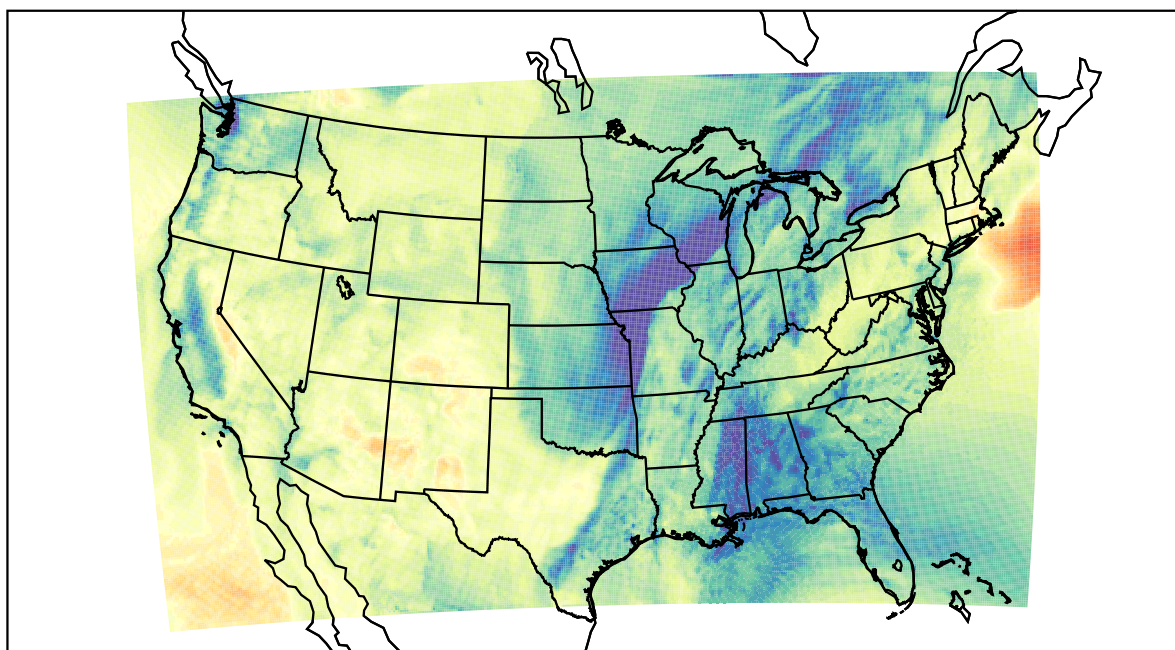
WRF (2020-11-10_18:00:00)
