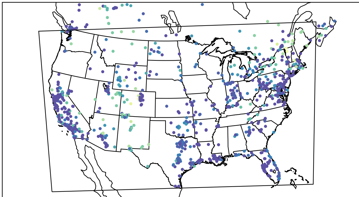
AirNOW (2020-11-10_08:00:00)
