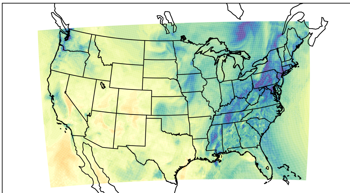
WRF (2020-11-11_20:00:00)
