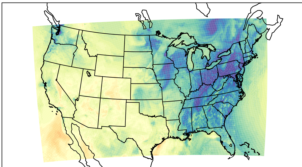
WRF (2020-11-11_22:00:00)
