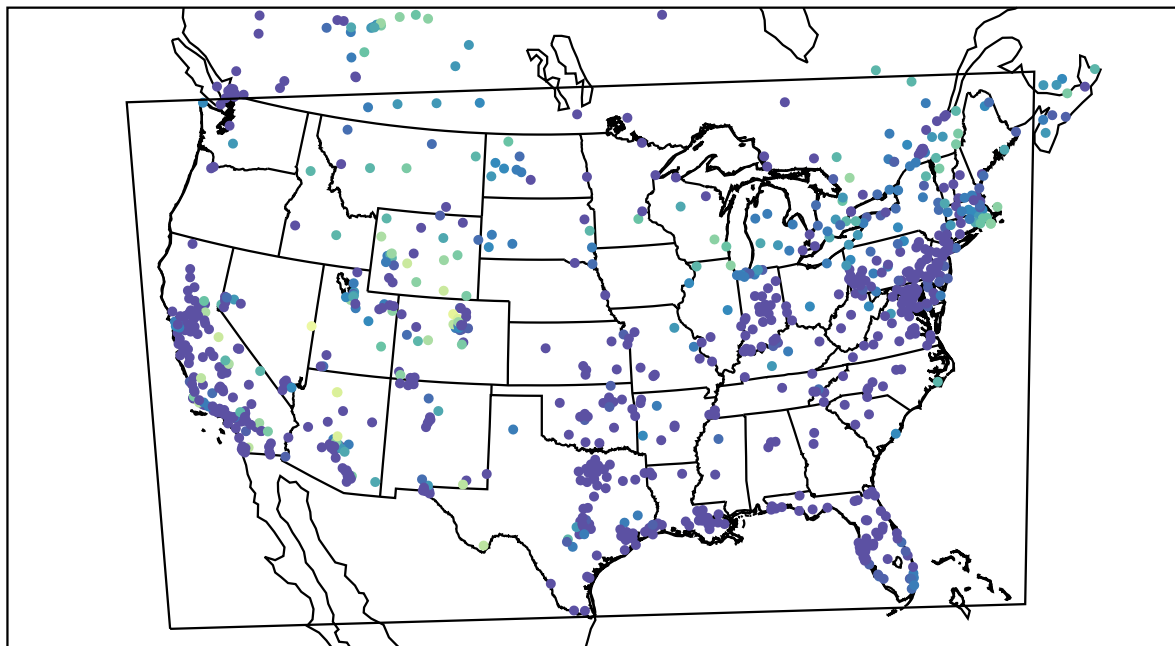
AirNOW (2020-11-11_14:00:00)
