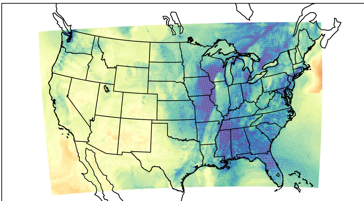
WRF (2020-11-10_23:00:00)
