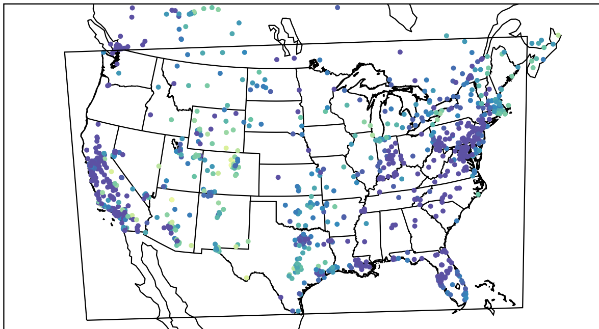
AirNOW (2020-11-11_16:00:00)
