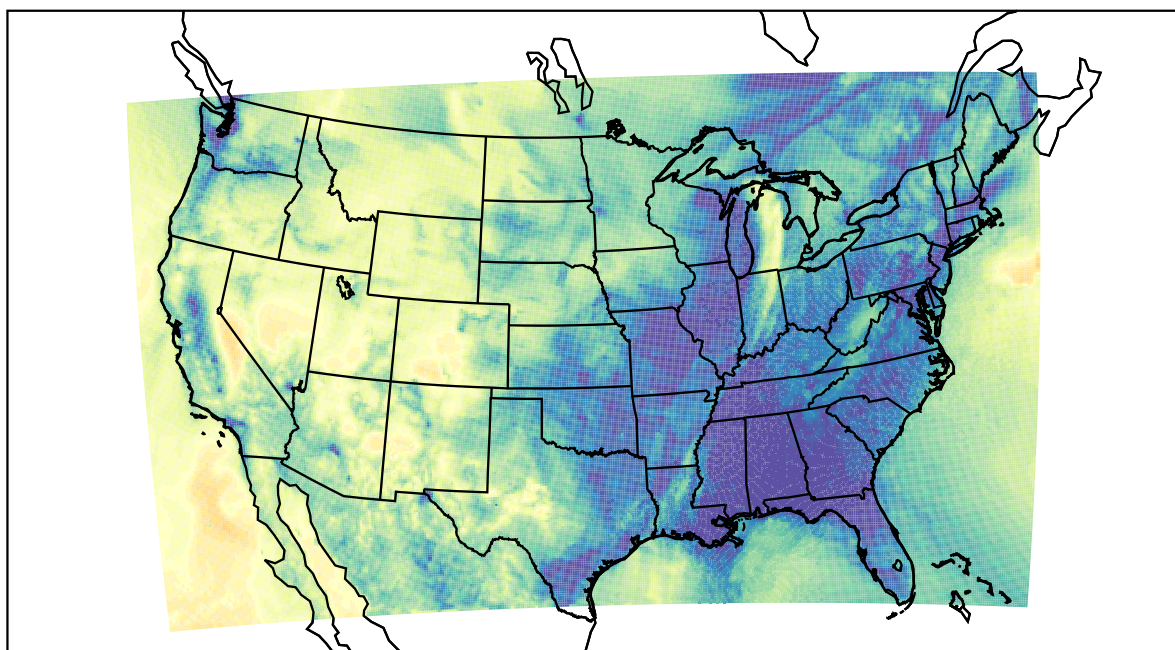
WRF (2020-11-11_06:00:00)
