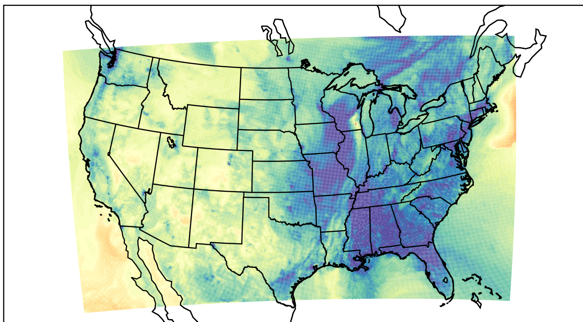
WRF (2020-11-11_01:00:00)
