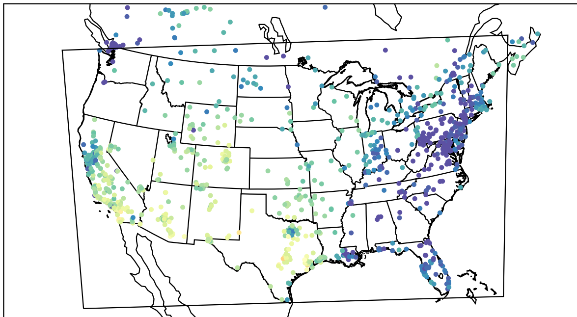
AirNOW (2020-11-11_20:00:00)
