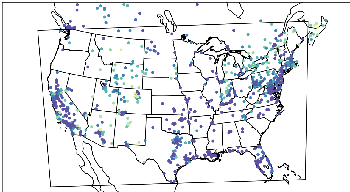
AirNOW (2020-11-11_04:00:00)
