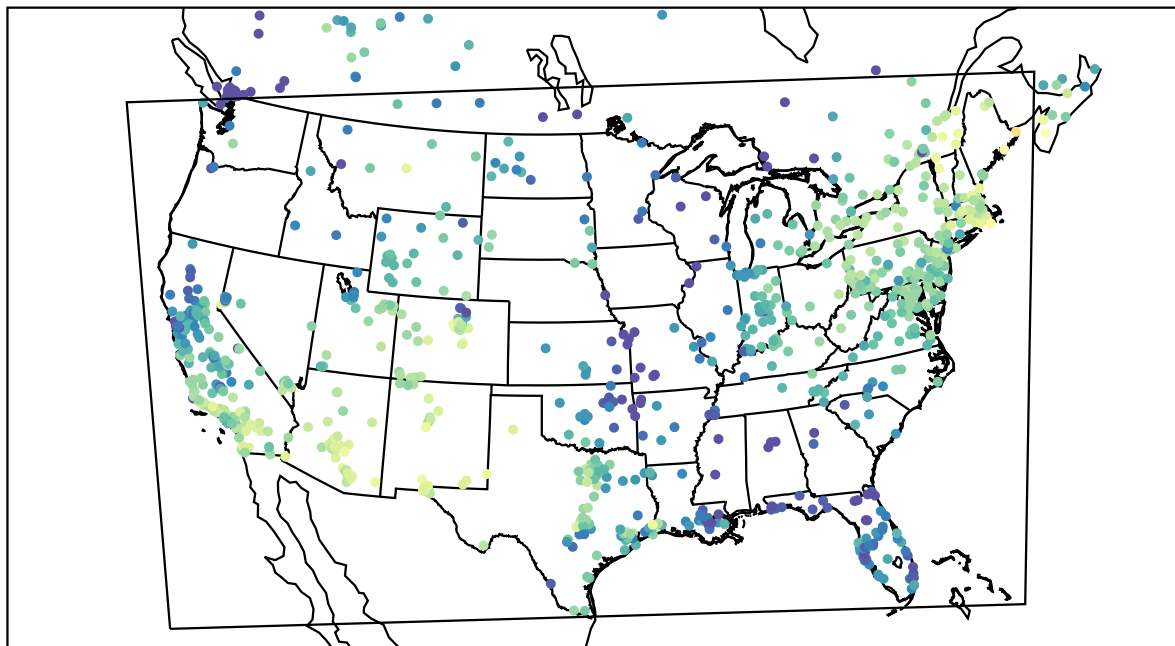
AirNOW (2020-11-10_19:00:00)
