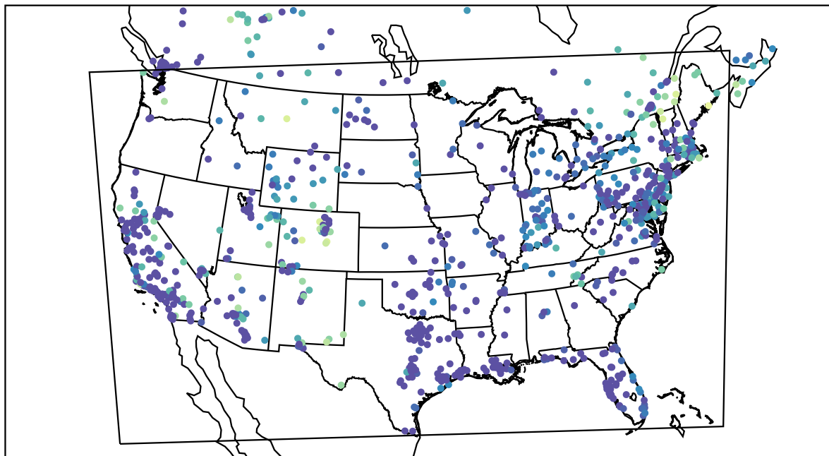
AirNOW (2020-11-10_14:00:00)
