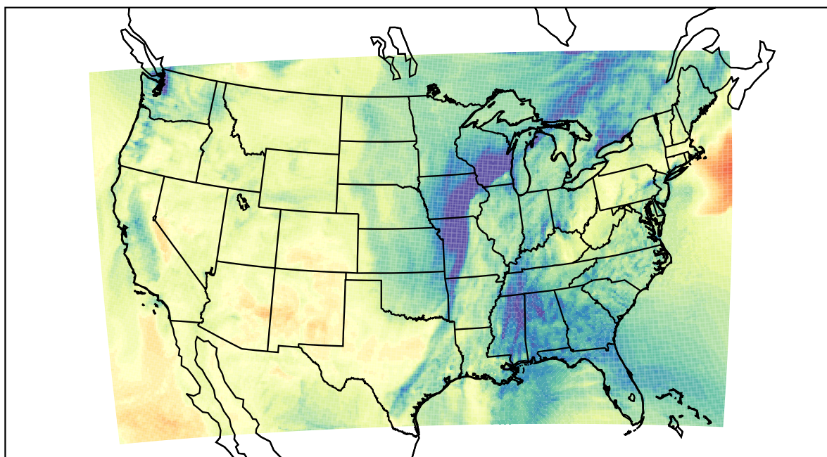
WRF (2020-11-10_20:00:00)
