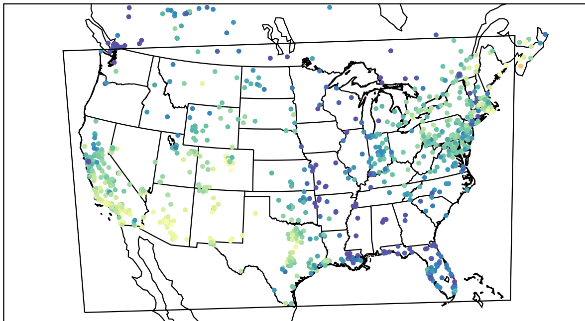
AirNOW (2020-11-10_21:00:00)
