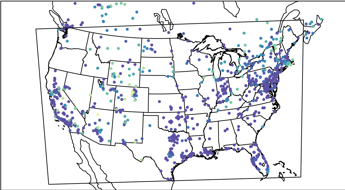
AirNOW (2020-11-11_11:00:00)
