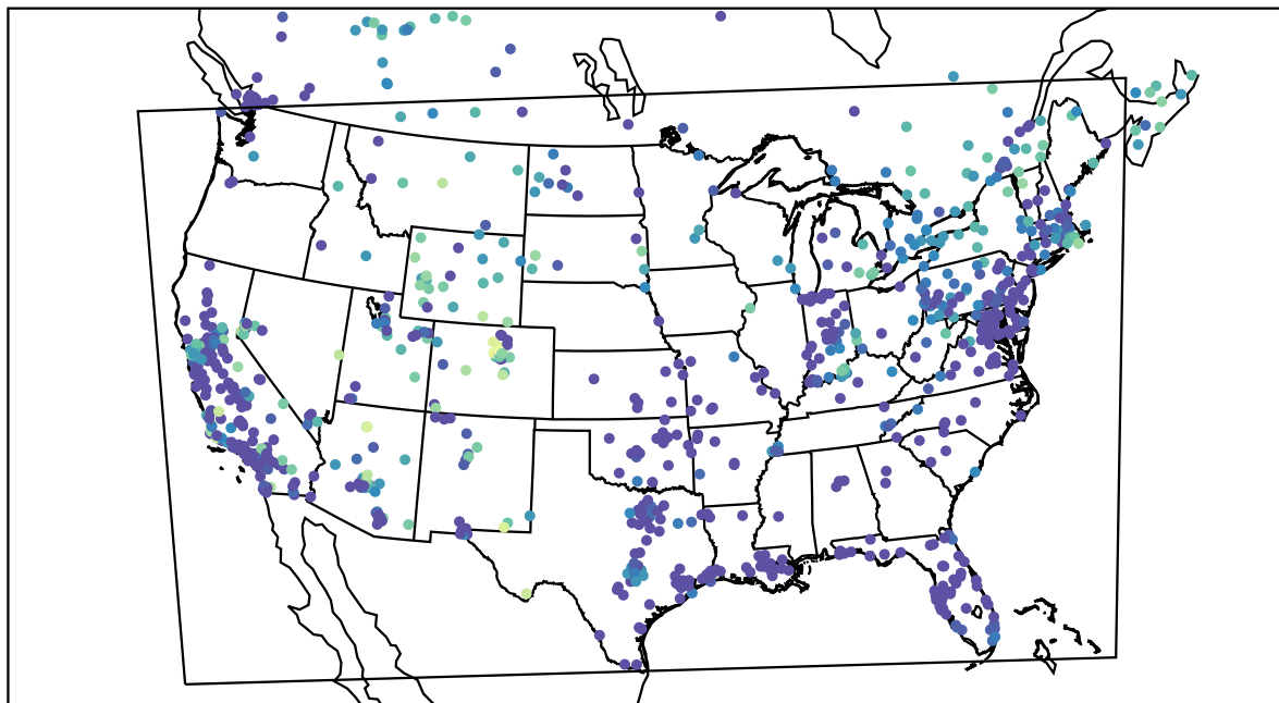
AirNOW (2020-11-11_08:00:00)
