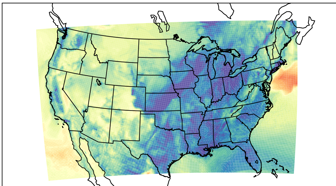
WRF (2020-11-10_08:00:00)
