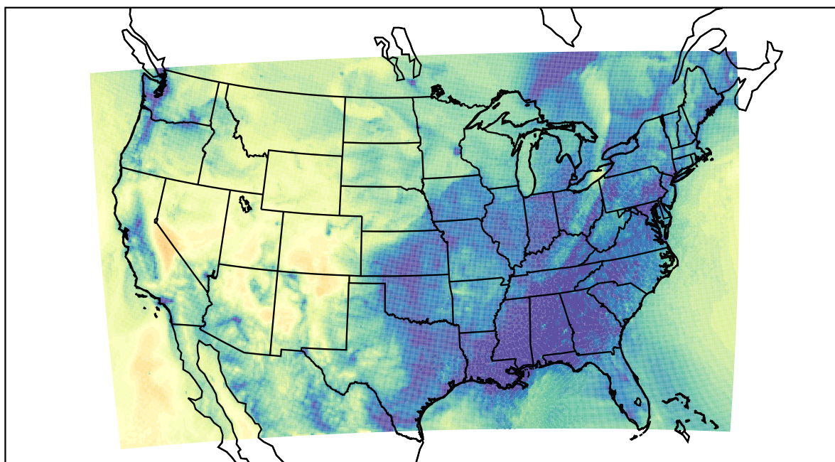
WRF (2020-11-11_14:00:00)
