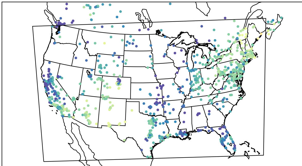
AirNOW (2020-11-10_18:00:00)
