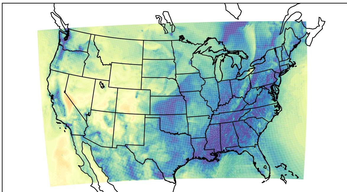
WRF (2020-11-11_15:00:00)
