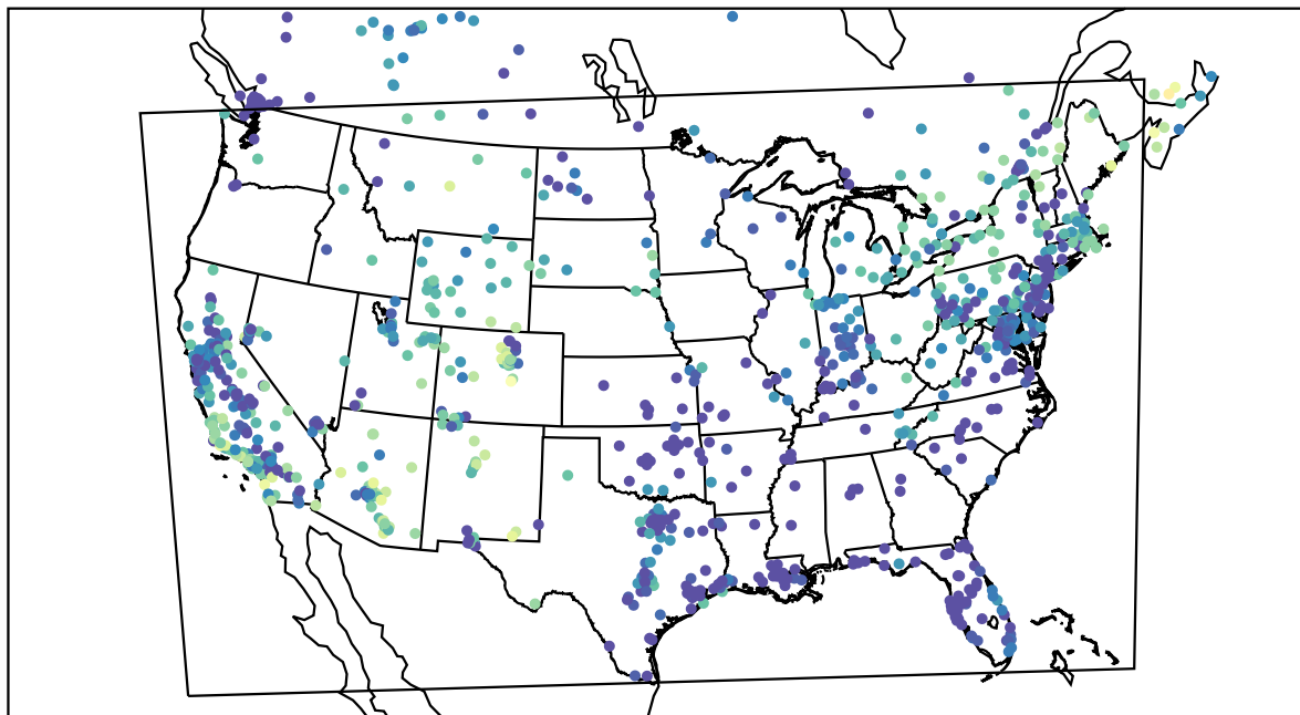
AirNOW (2020-11-11_01:00:00)
