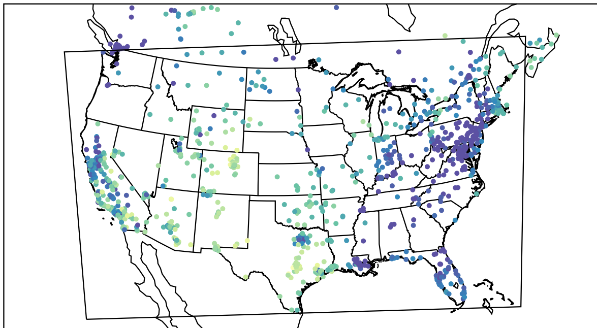
AirNOW (2020-11-11_18:00:00)
