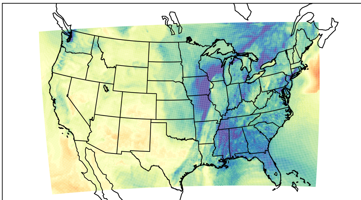
WRF (2020-11-10_22:00:00)
