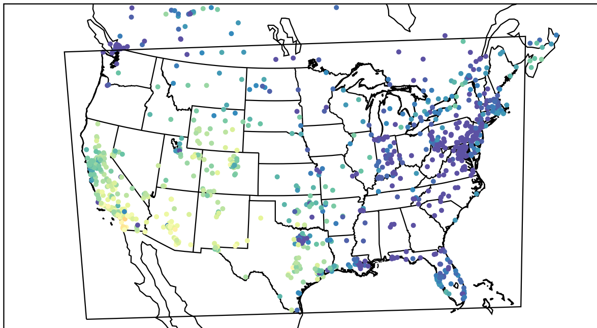
AirNOW (2020-11-11_23:00:00)
