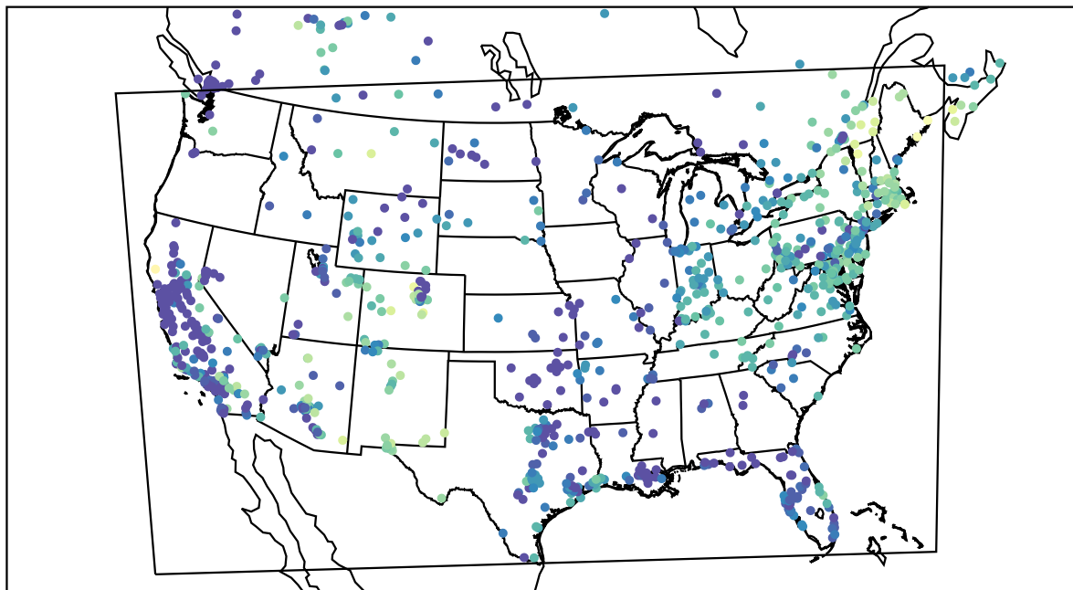
AirNOW (2020-11-10_16:00:00)
