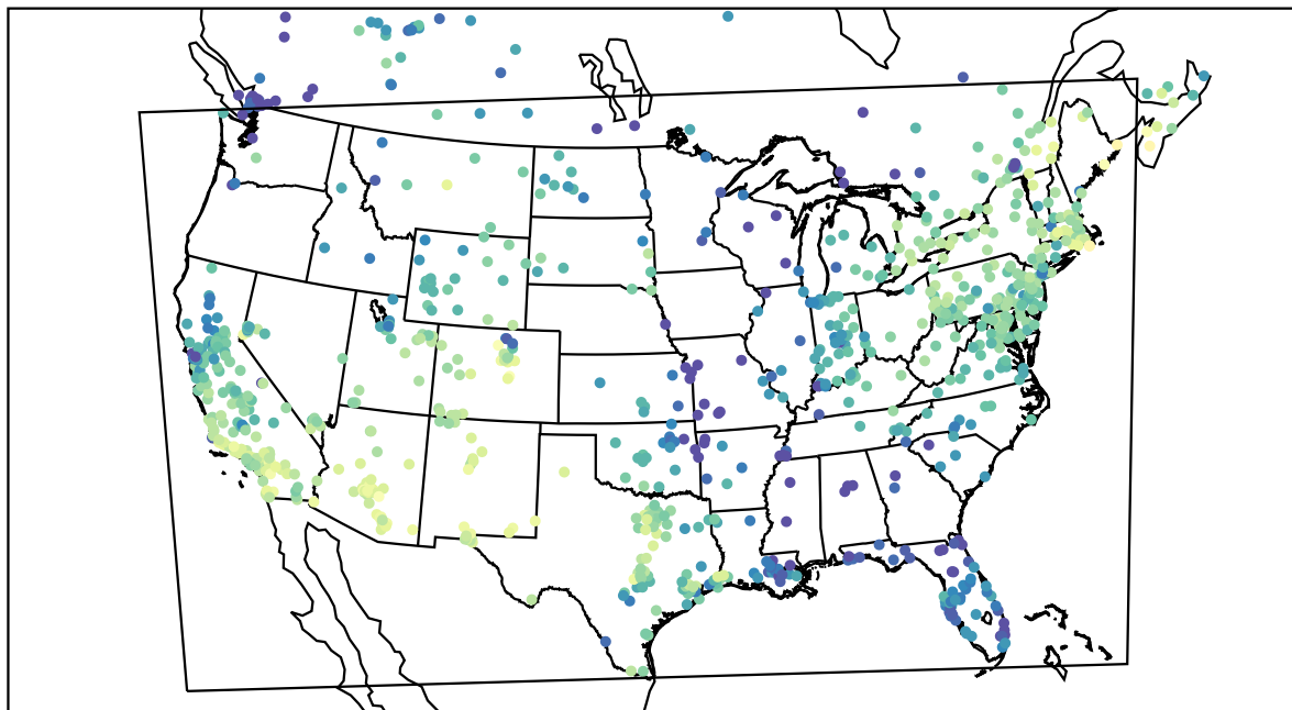
AirNOW (2020-11-10_20:00:00)
