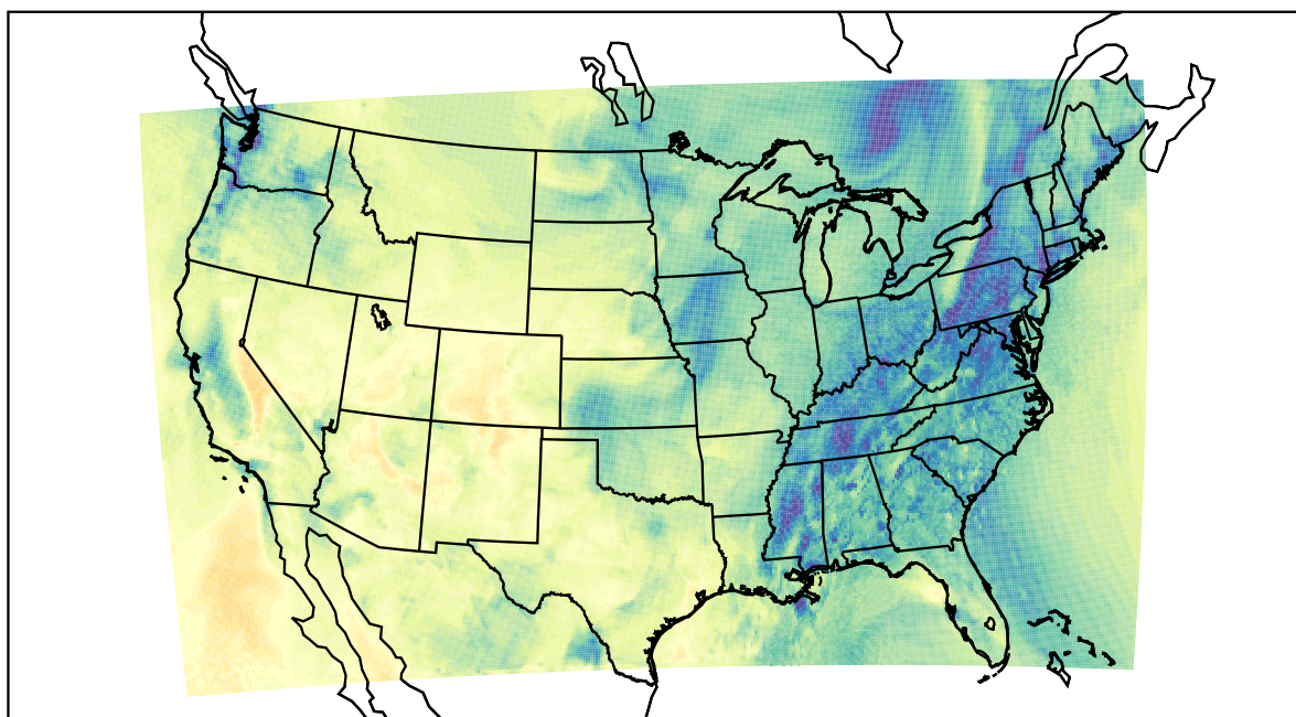
WRF (2020-11-11_19:00:00)
