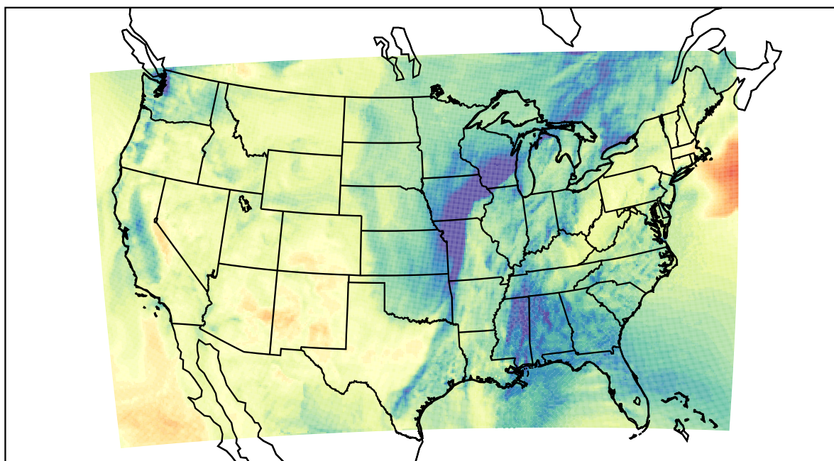
WRF (2020-11-10_19:00:00)
