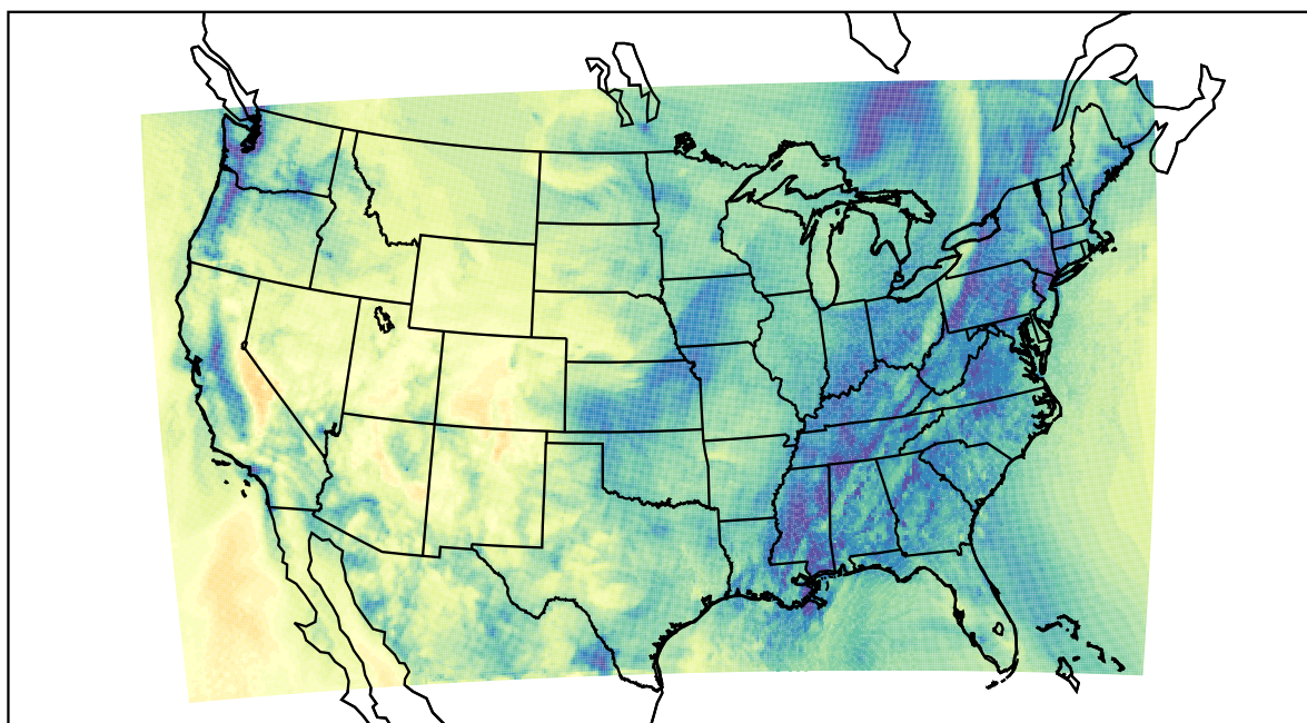
WRF (2020-11-11_17:00:00)
