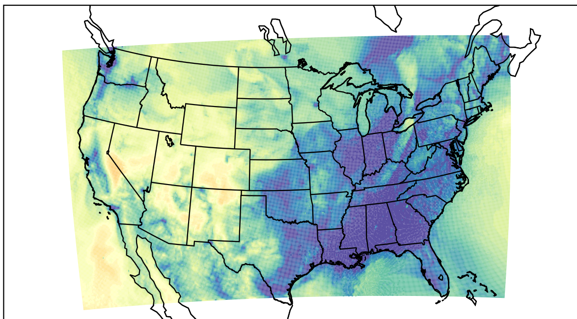
WRF (2020-11-11_13:00:00)
