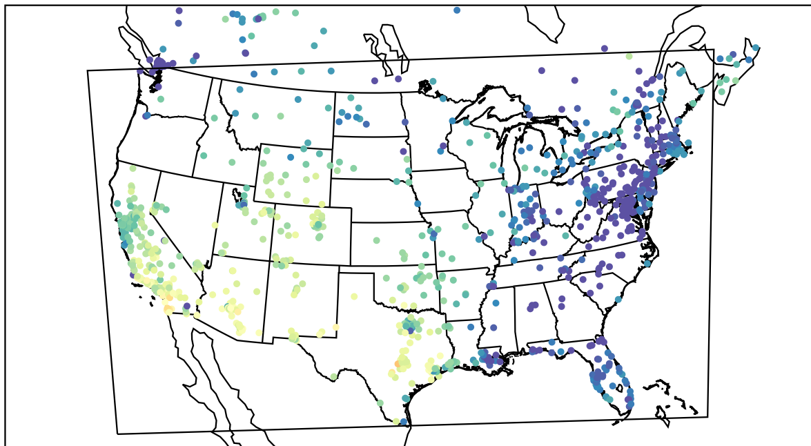
AirNOW (2020-11-11_22:00:00)
