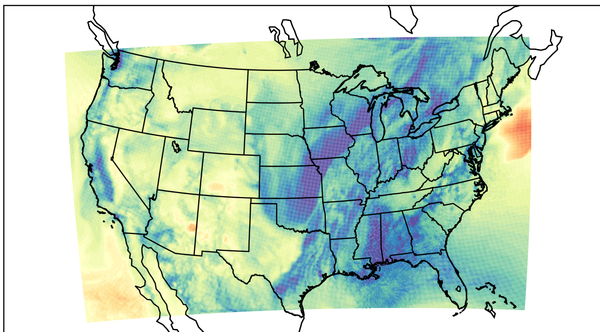
WRF (2020-11-10_16:00:00)
