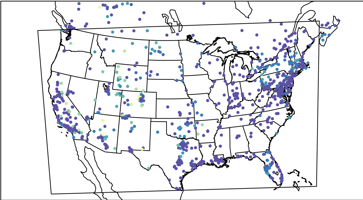
AirNOW (2020-11-12_11:00:00)
