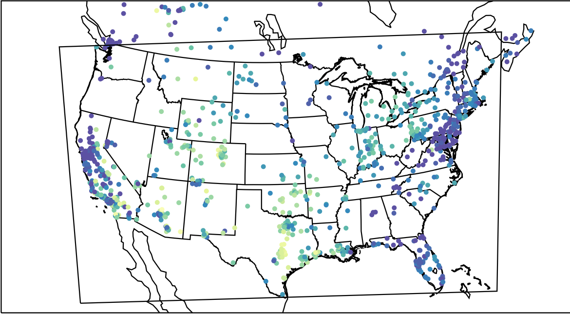
AirNOW (2020-11-12_17:00:00)
