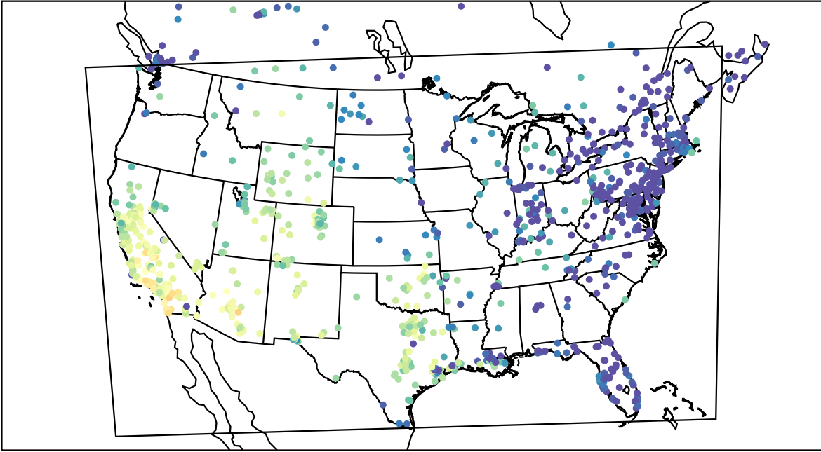
AirNOW (2020-11-12_23:00:00)
