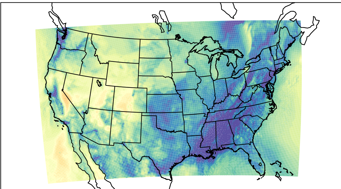
WRF (2020-11-11_15:00:00)
