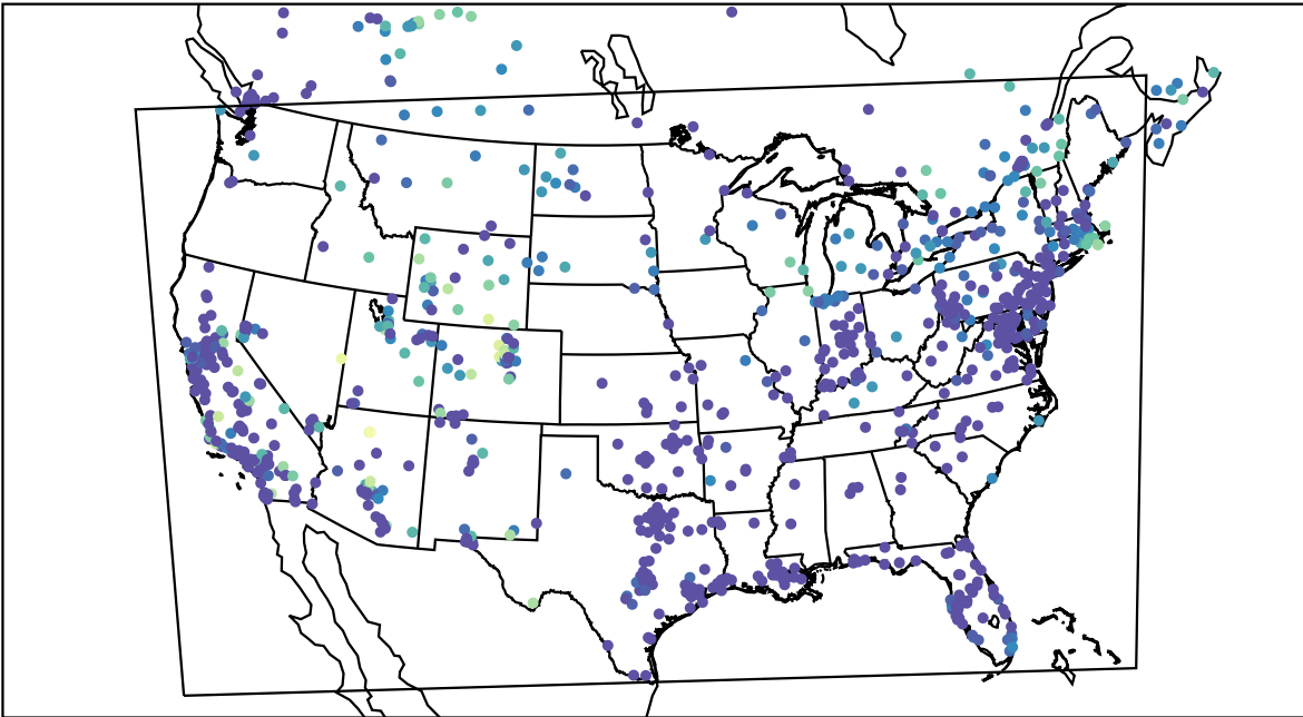
AirNOW (2020-11-11_13:00:00)
