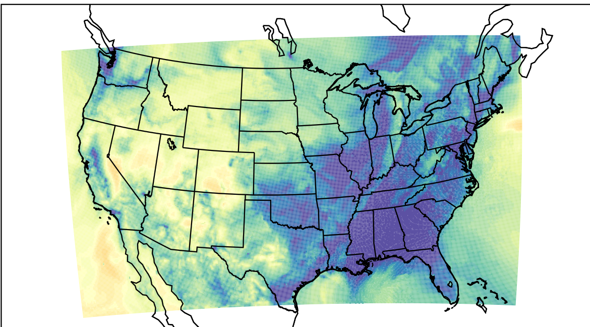
WRF (2020-11-11_08:00:00)
