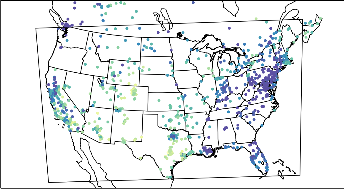
AirNOW (2020-11-11_18:00:00)
