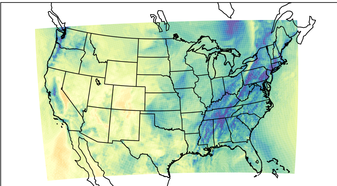
WRF (2020-11-11_18:00:00)
