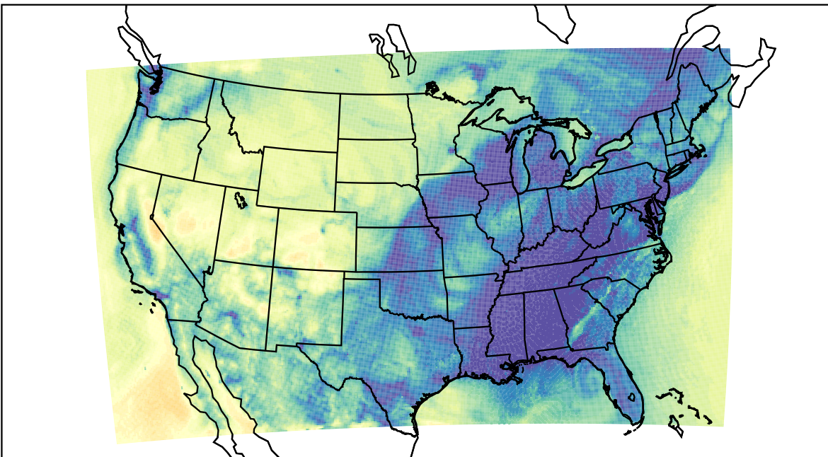
WRF (2020-11-12_13:00:00)
