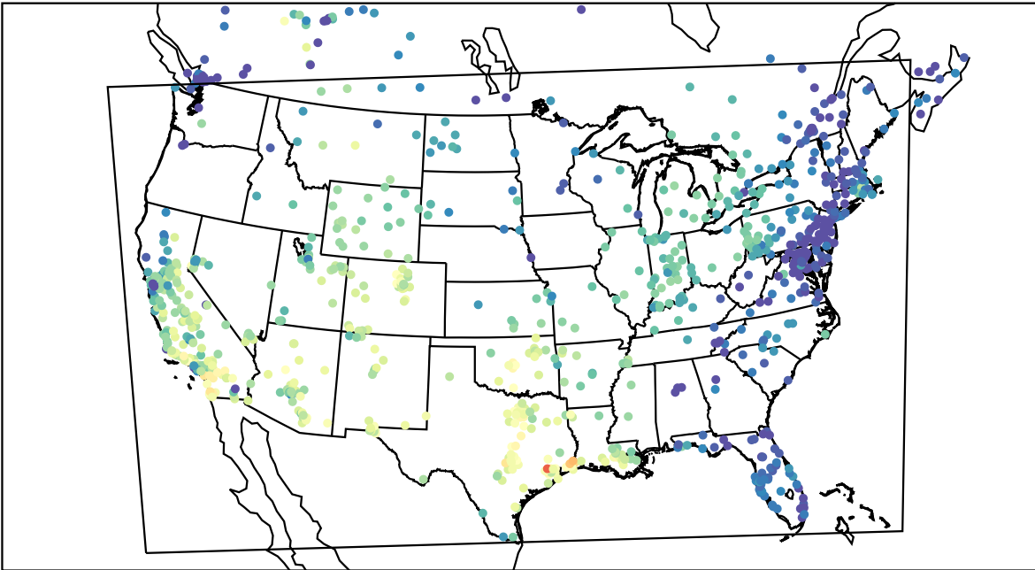
AirNOW (2020-11-12_19:00:00)
