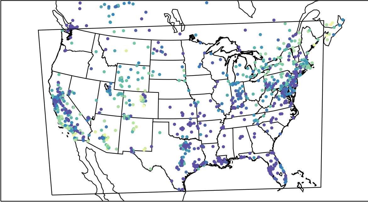
AirNOW (2020-11-11_01:00:00)
