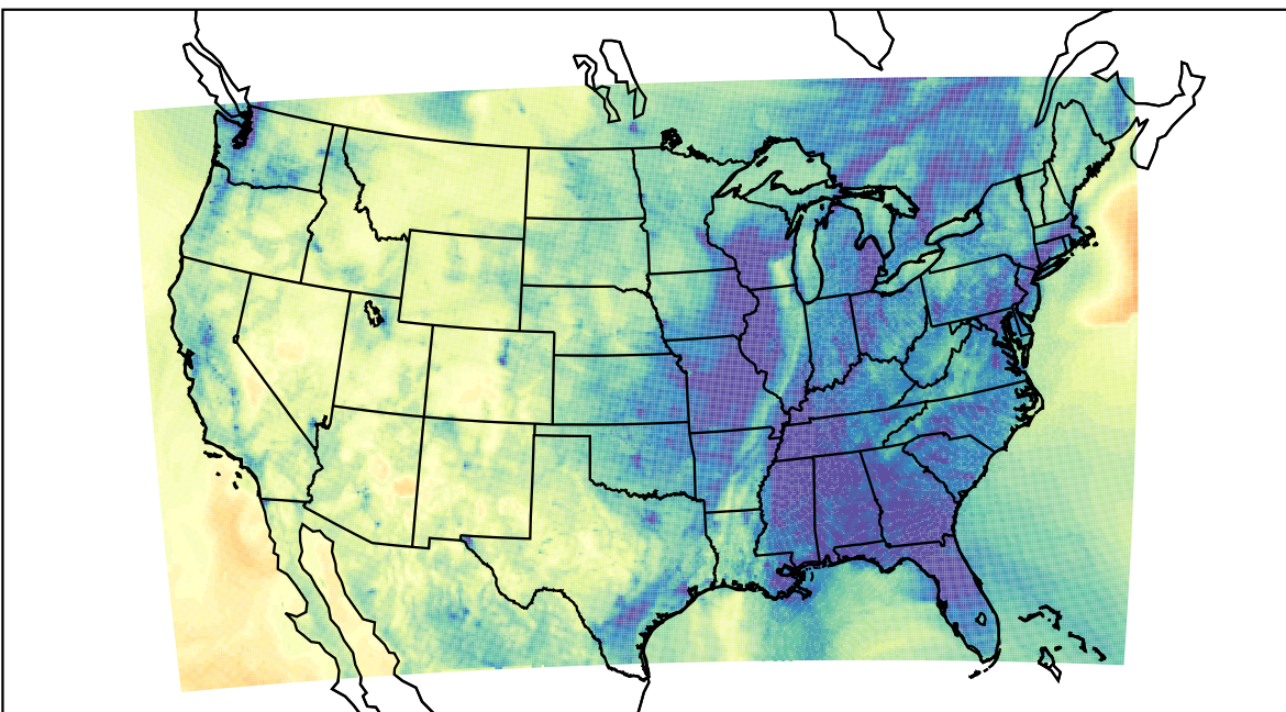
WRF (2020-11-11_01:00:00)
