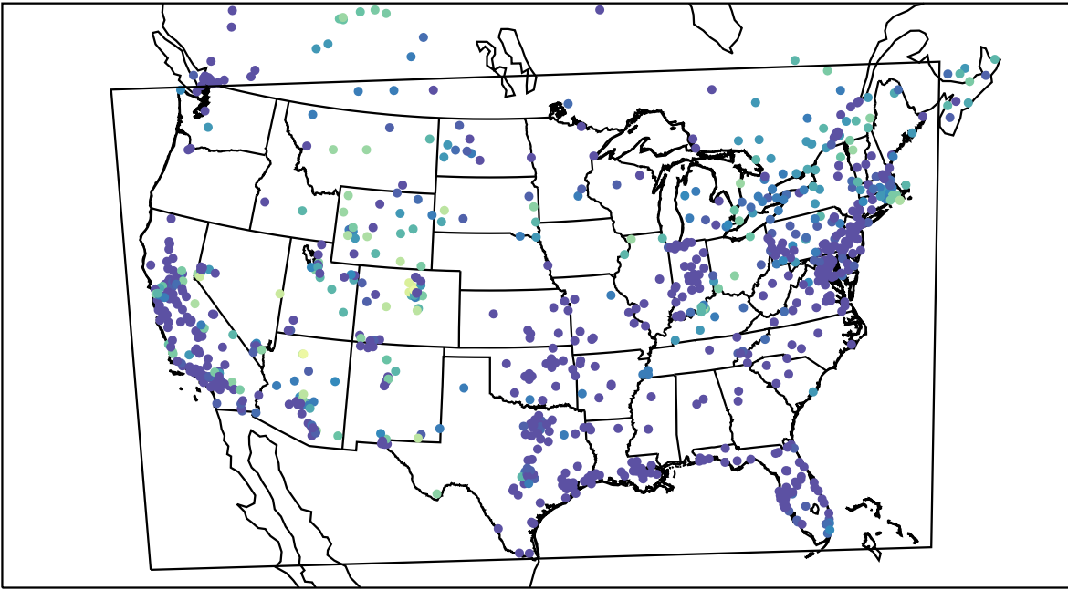
AirNOW (2020-11-11_10:00:00)
