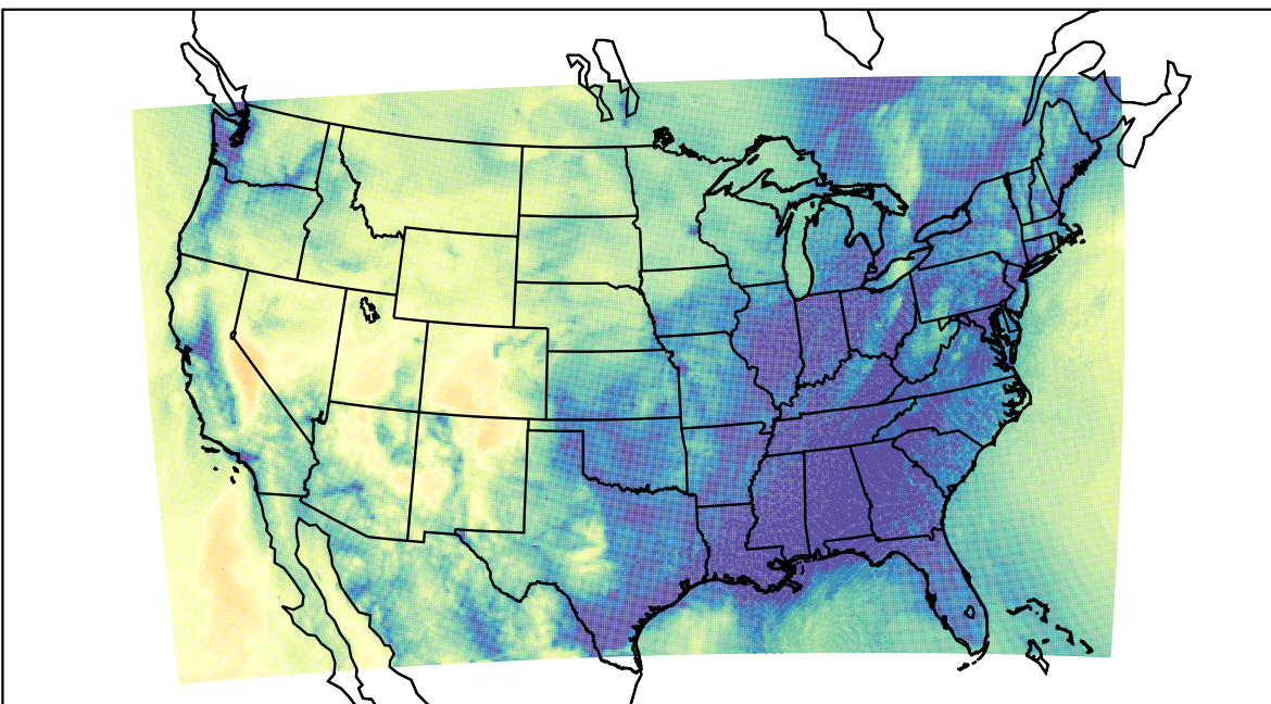
WRF (2020-11-11_13:00:00)
