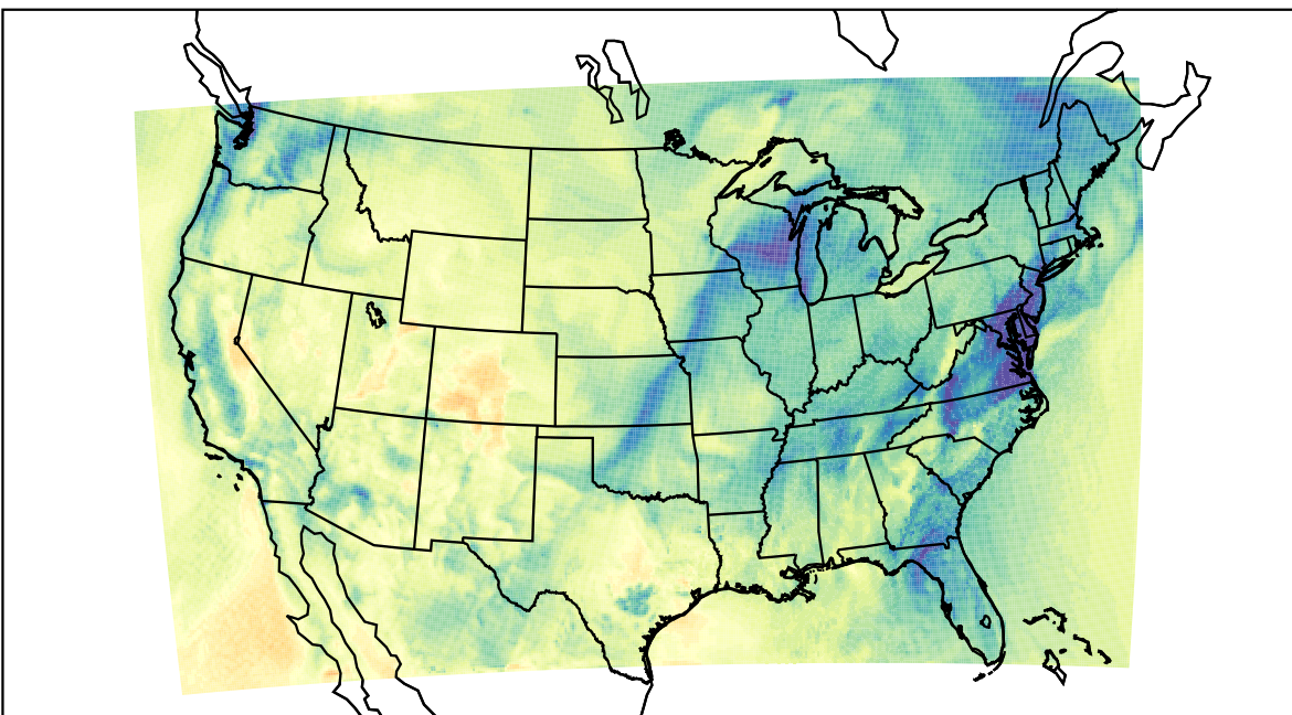
WRF (2020-11-12_18:00:00)
