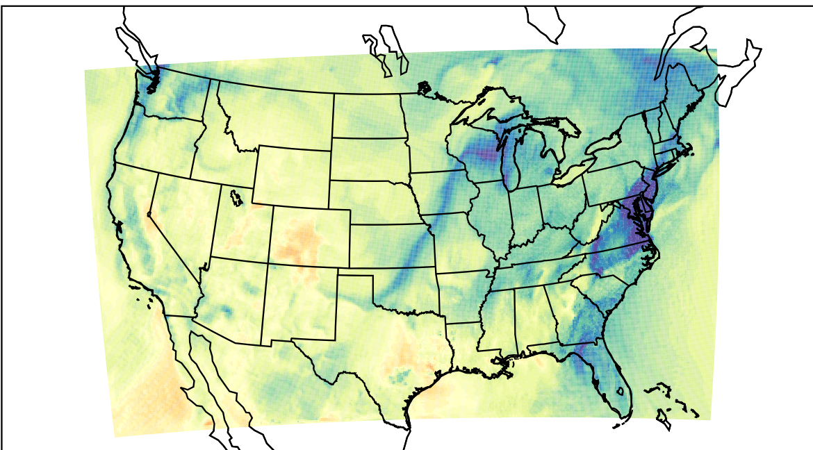
WRF (2020-11-12_19:00:00)
