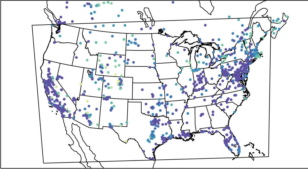
AirNOW (2020-11-11_15:00:00)
