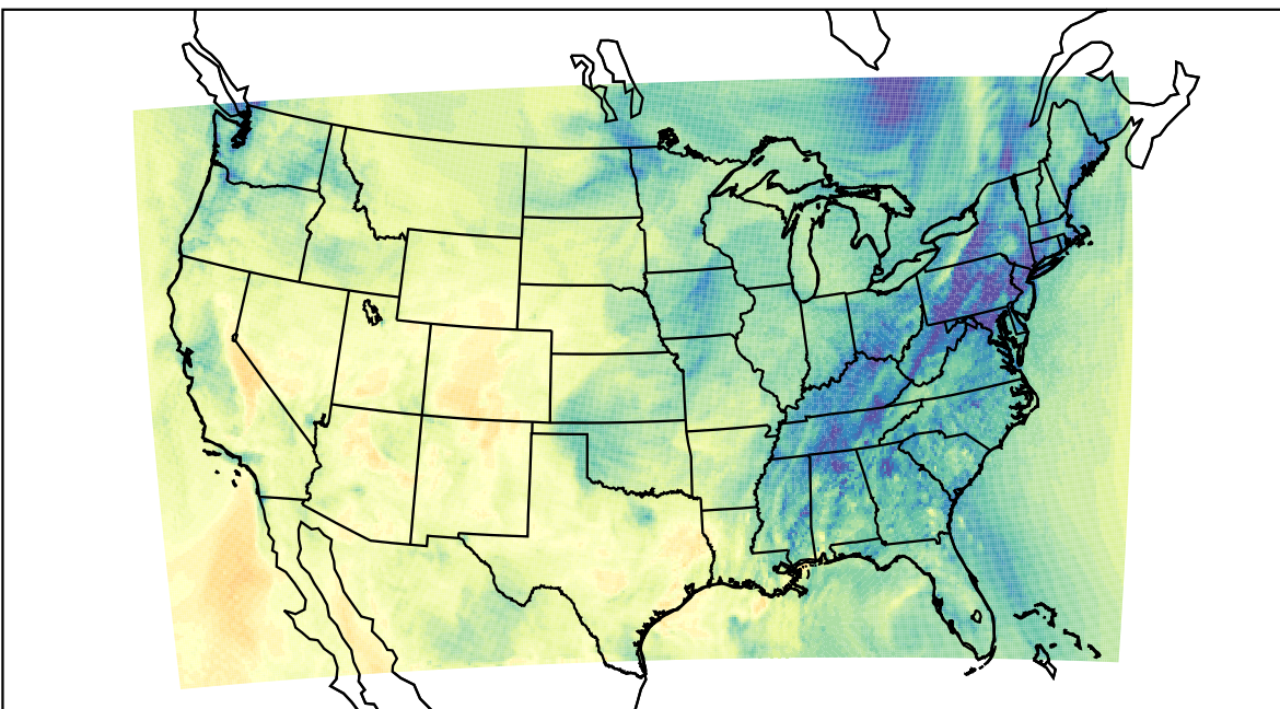
WRF (2020-11-11_20:00:00)
