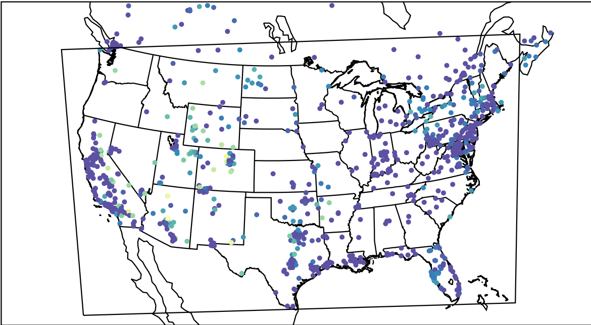
AirNOW (2020-11-12_10:00:00)
