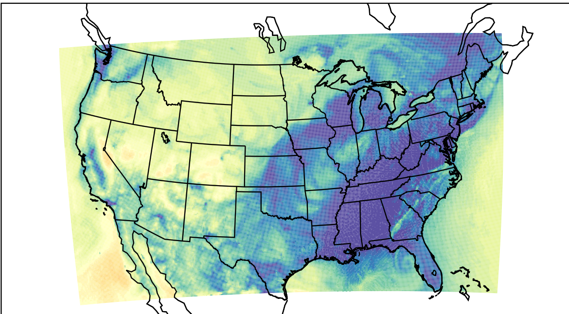
WRF (2020-11-12_12:00:00)
