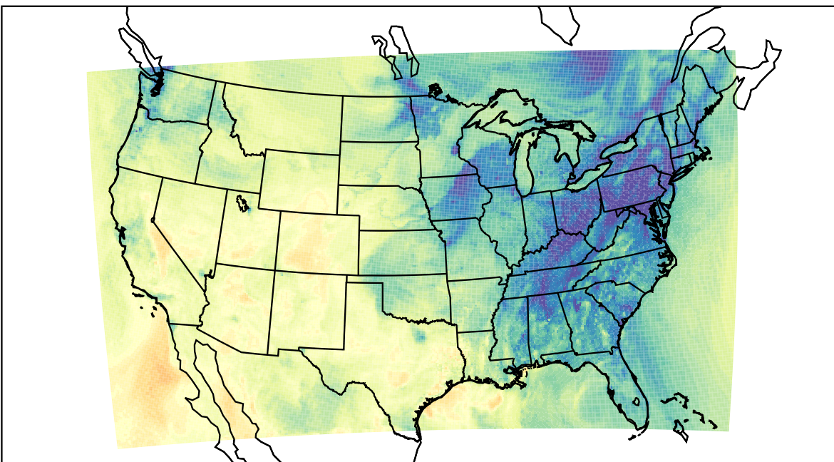
WRF (2020-11-11_22:00:00)
