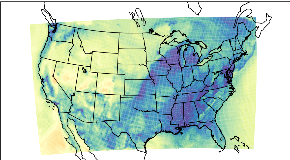
WRF (2020-11-12_15:00:00)
