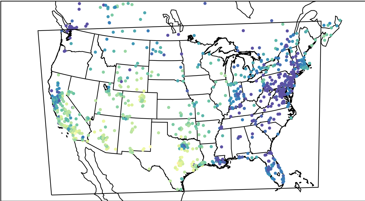
AirNOW (2020-11-11_19:00:00)
