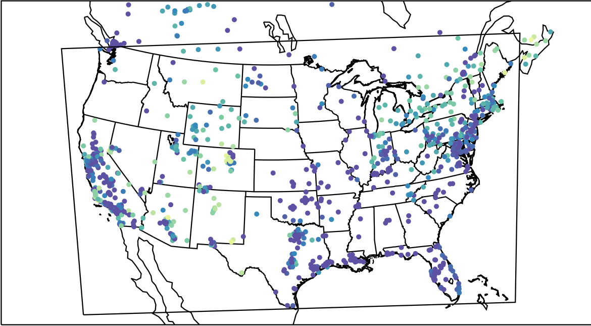
AirNOW (2020-11-11_03:00:00)
