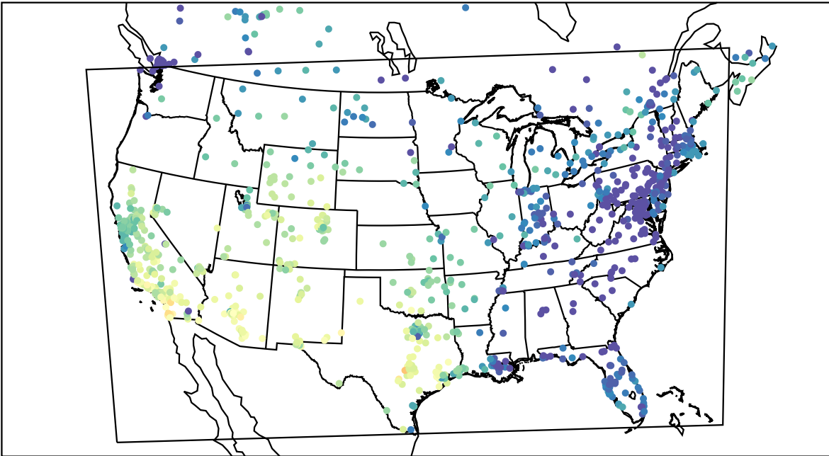
AirNOW (2020-11-11_22:00:00)
