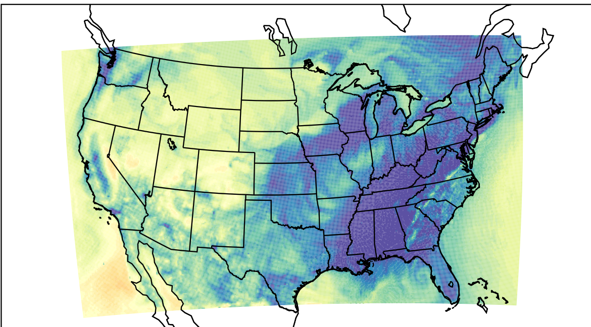
WRF (2020-11-12_10:00:00)
