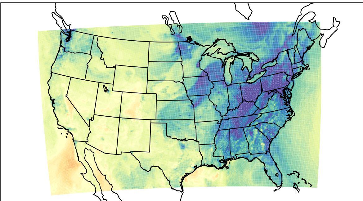
WRF (2020-11-11_23:00:00)
