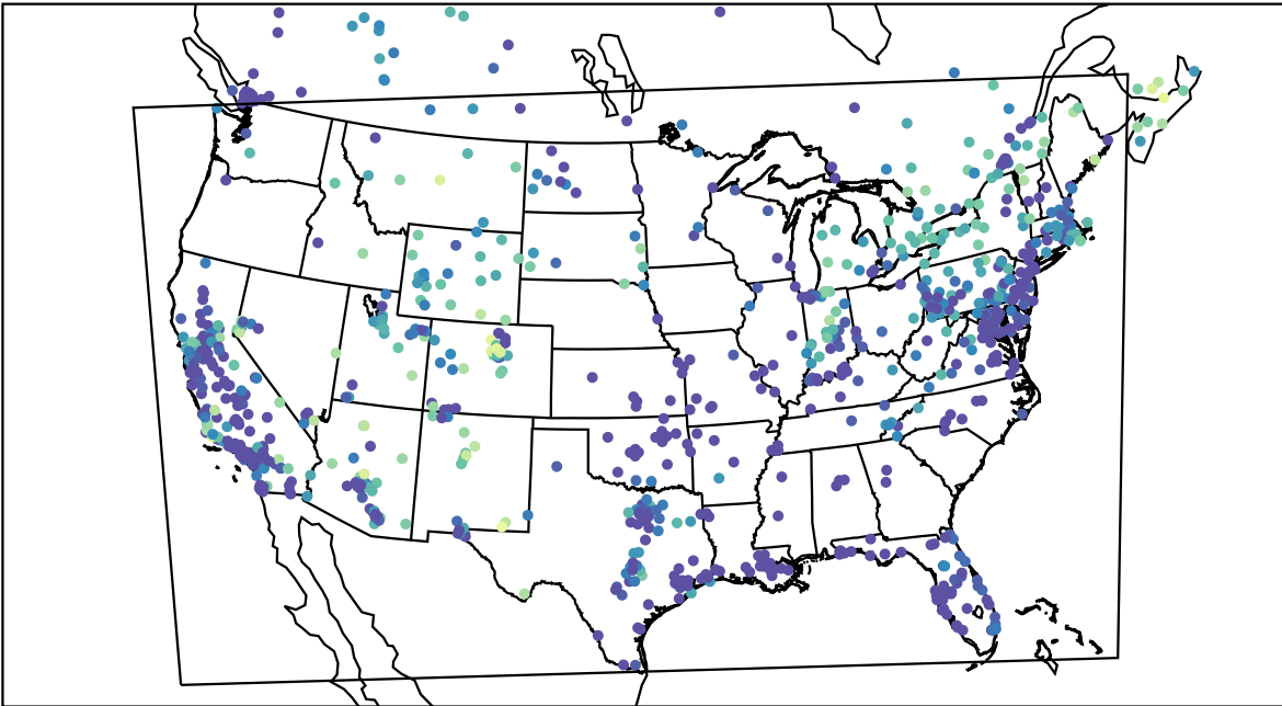
AirNOW (2020-11-11_04:00:00)
