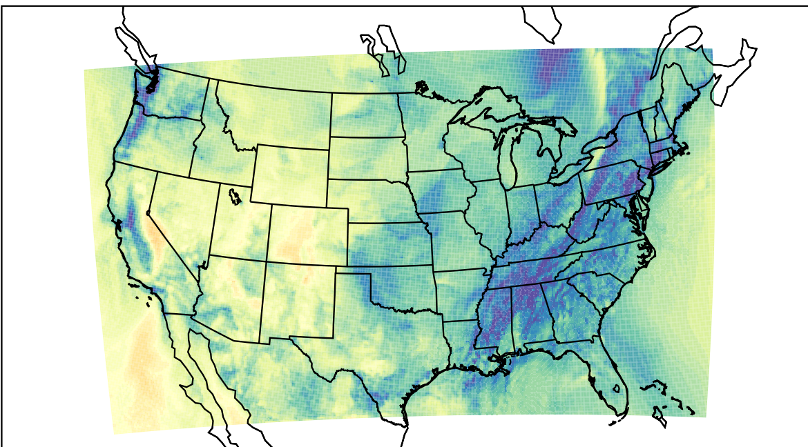
WRF (2020-11-11_17:00:00)
