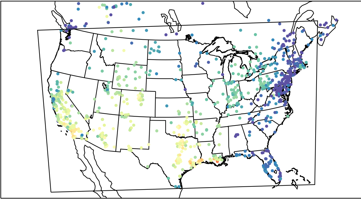
AirNOW (2020-11-12_20:00:00)
