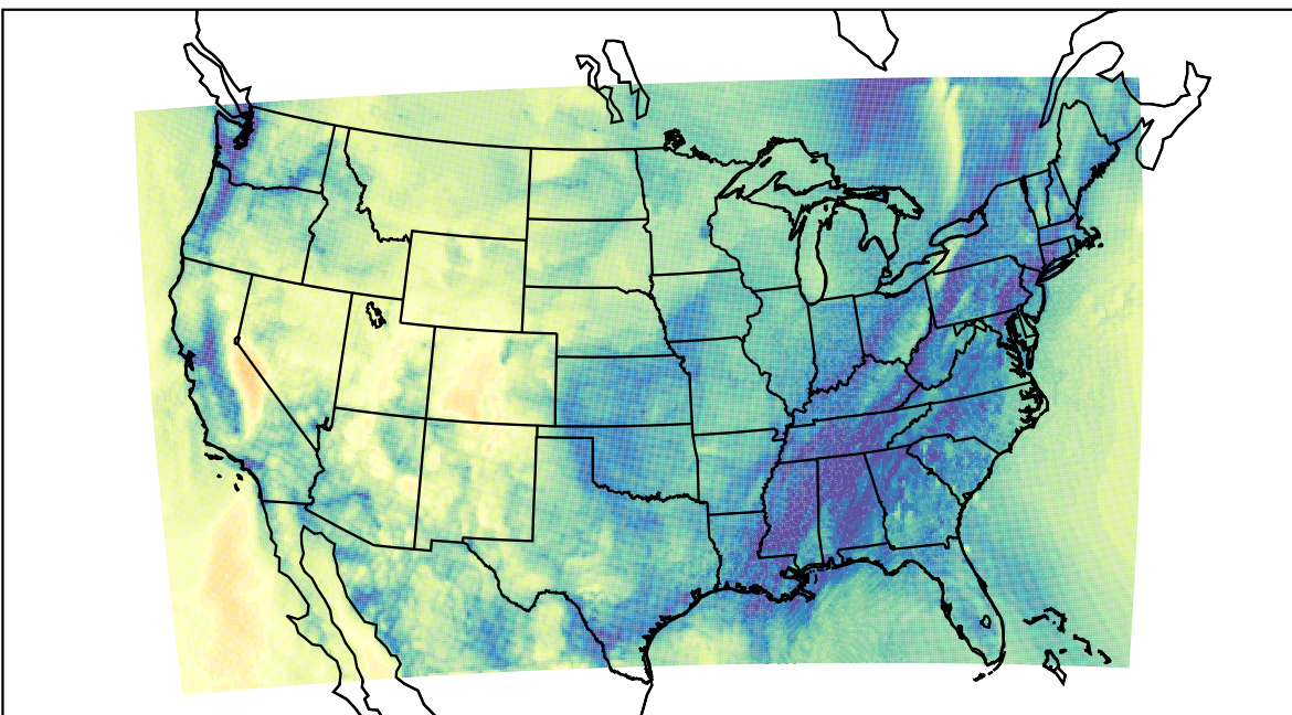
WRF (2020-11-11_16:00:00)
