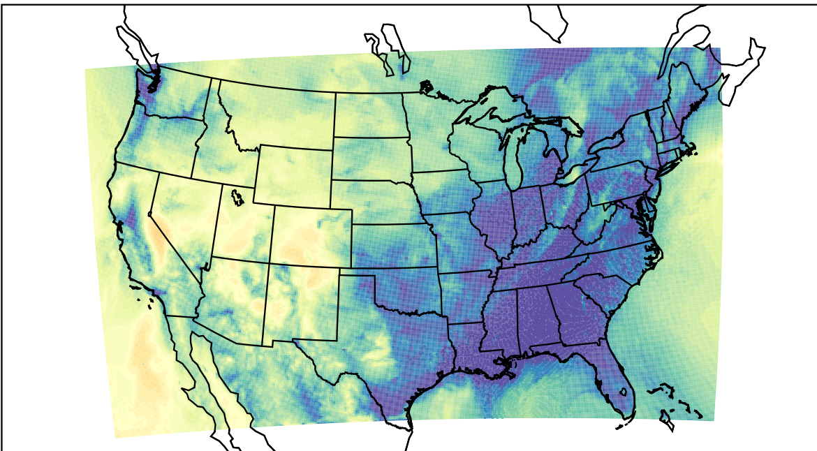
WRF (2020-11-11_12:00:00)
