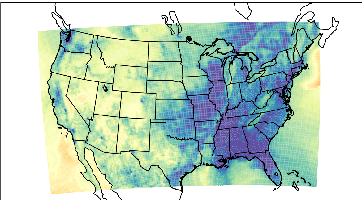
WRF (2020-11-11_03:00:00)
