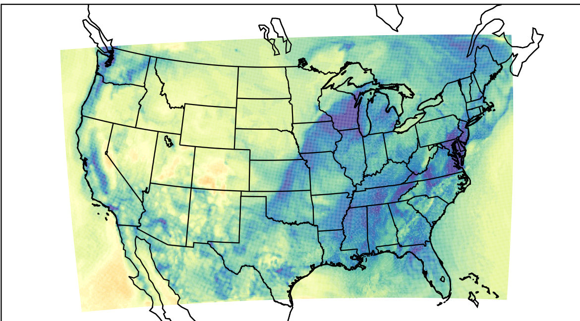
WRF (2020-11-12_16:00:00)
