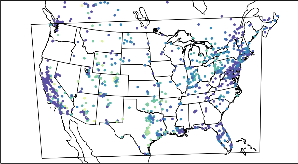
AirNOW (2020-11-12_16:00:00)
