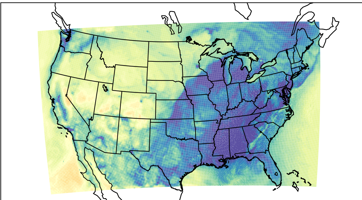
WRF (2020-11-12_14:00:00)
