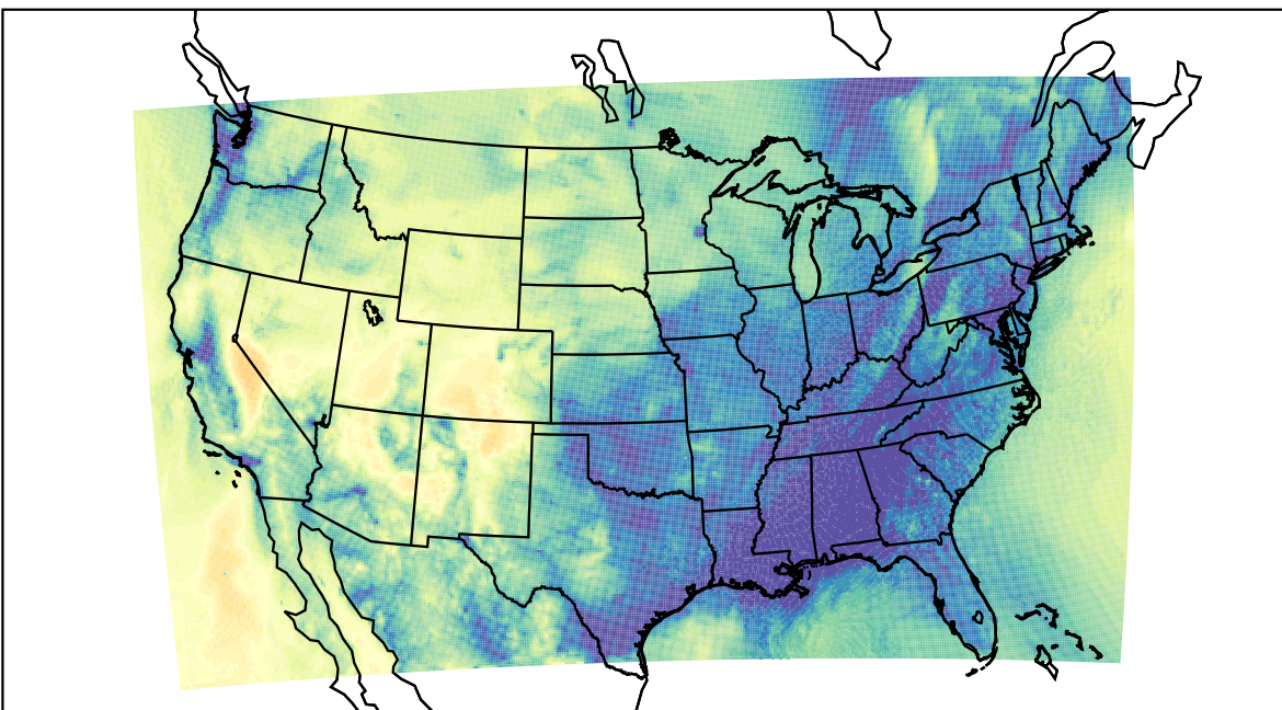
WRF (2020-11-11_14:00:00)
