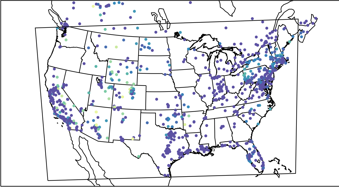
AirNOW (2020-11-12_13:00:00)
