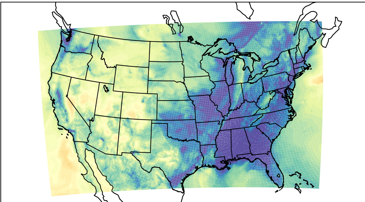
WRF (2020-11-11_06:00:00)
