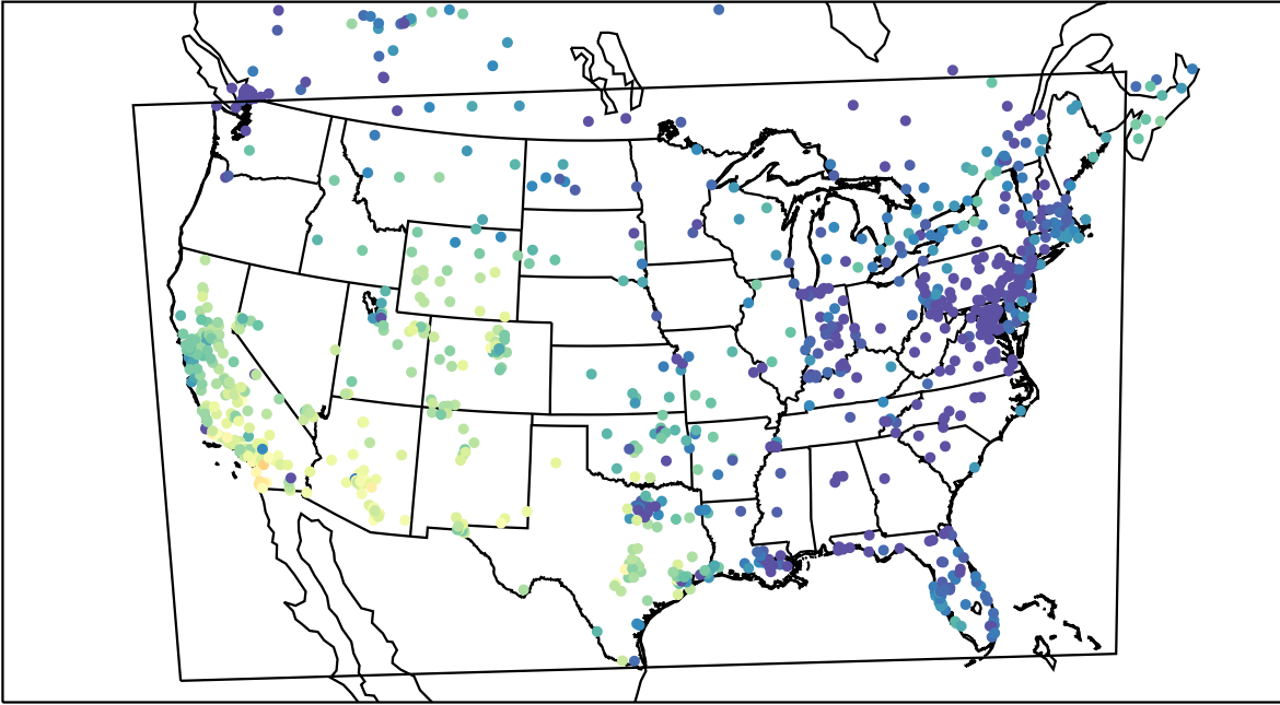
AirNOW (2020-11-11_23:00:00)
