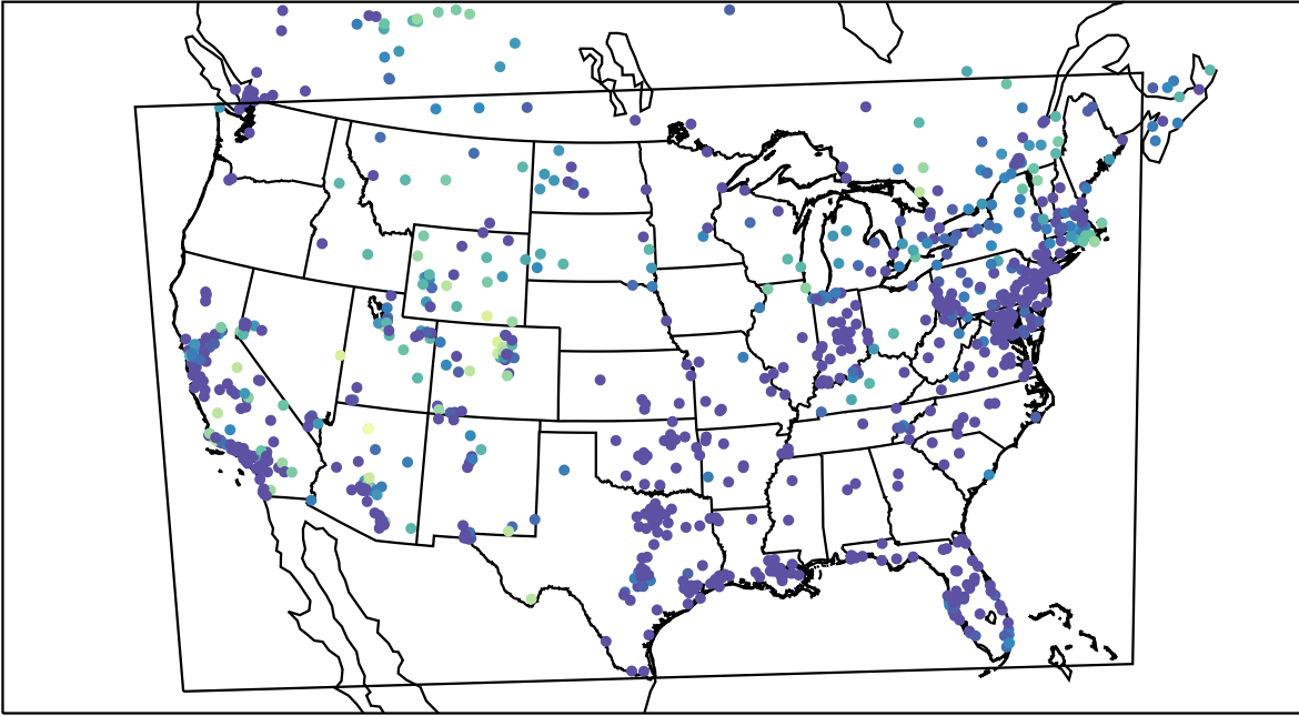
AirNOW (2020-11-11_12:00:00)
