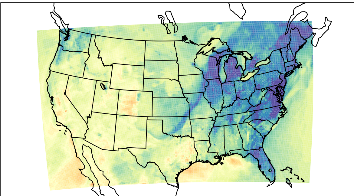
WRF (2020-11-12_23:00:00)
