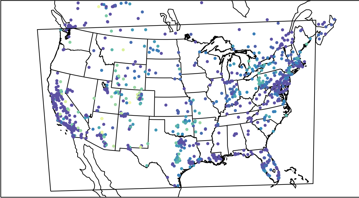
AirNOW (2020-11-12_15:00:00)
