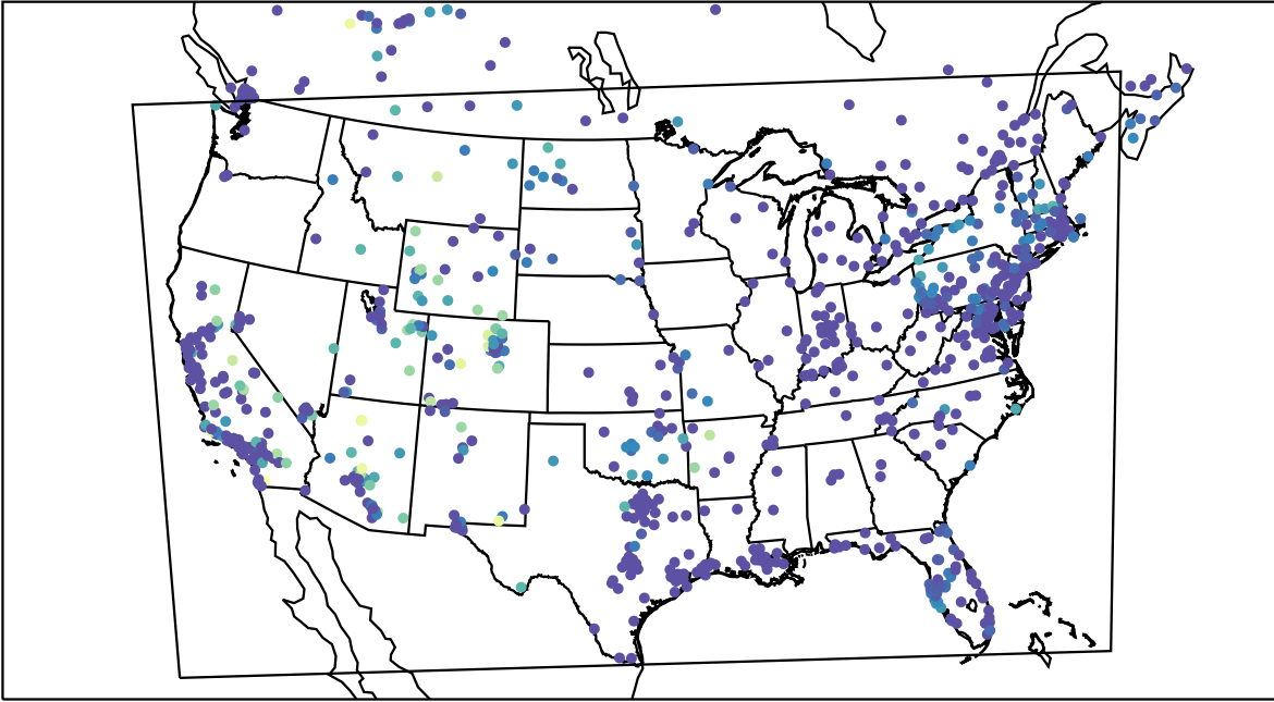
AirNOW (2020-11-12_12:00:00)
