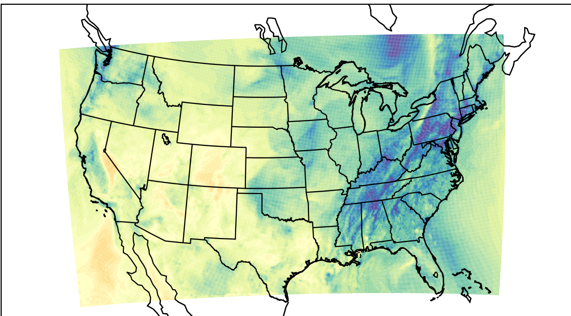
WRF (2020-11-11_19:00:00)
