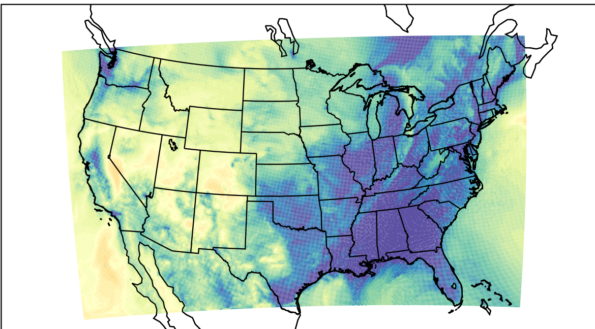
WRF (2020-11-11_10:00:00)
