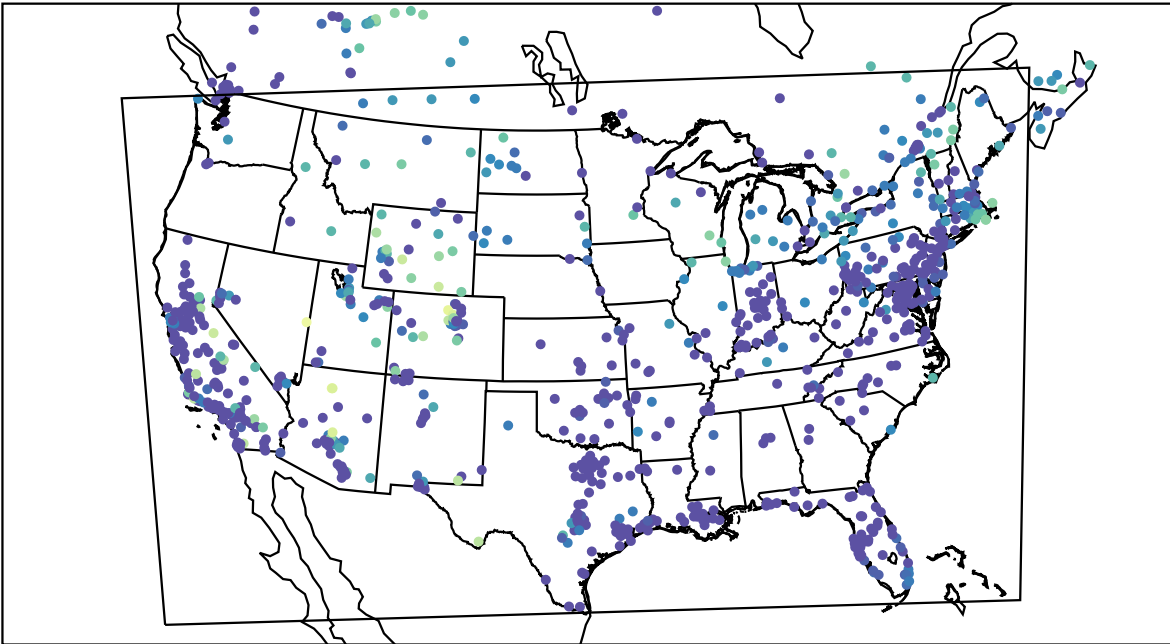
AirNOW (2020-11-11_14:00:00)
