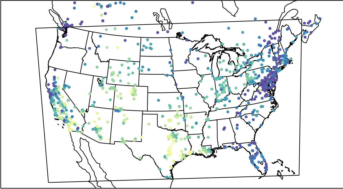
AirNOW (2020-11-12_18:00:00)
