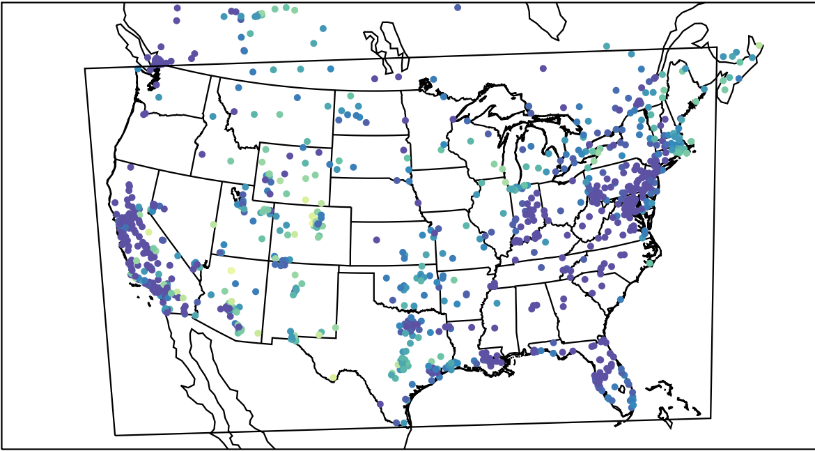
AirNOW (2020-11-11_16:00:00)
