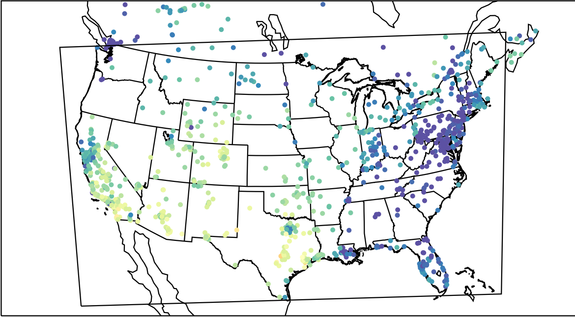
AirNOW (2020-11-11_20:00:00)
