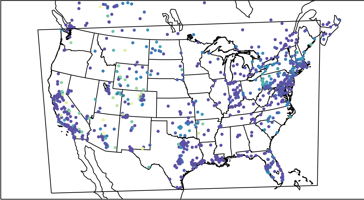
AirNOW (2020-11-12_14:00:00)
