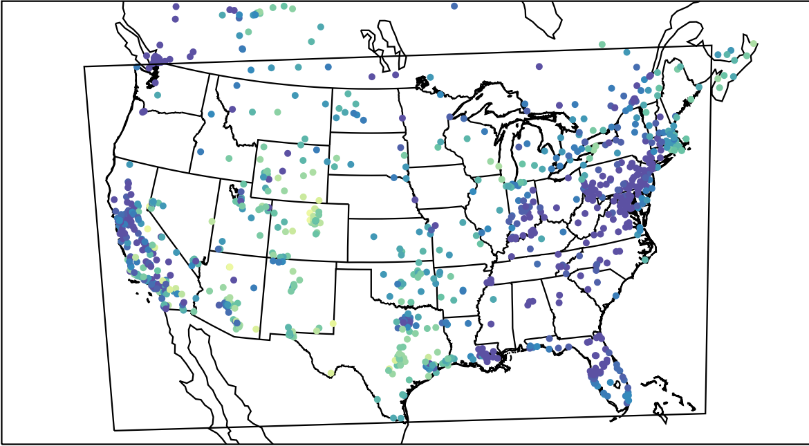
AirNOW (2020-11-11_17:00:00)
