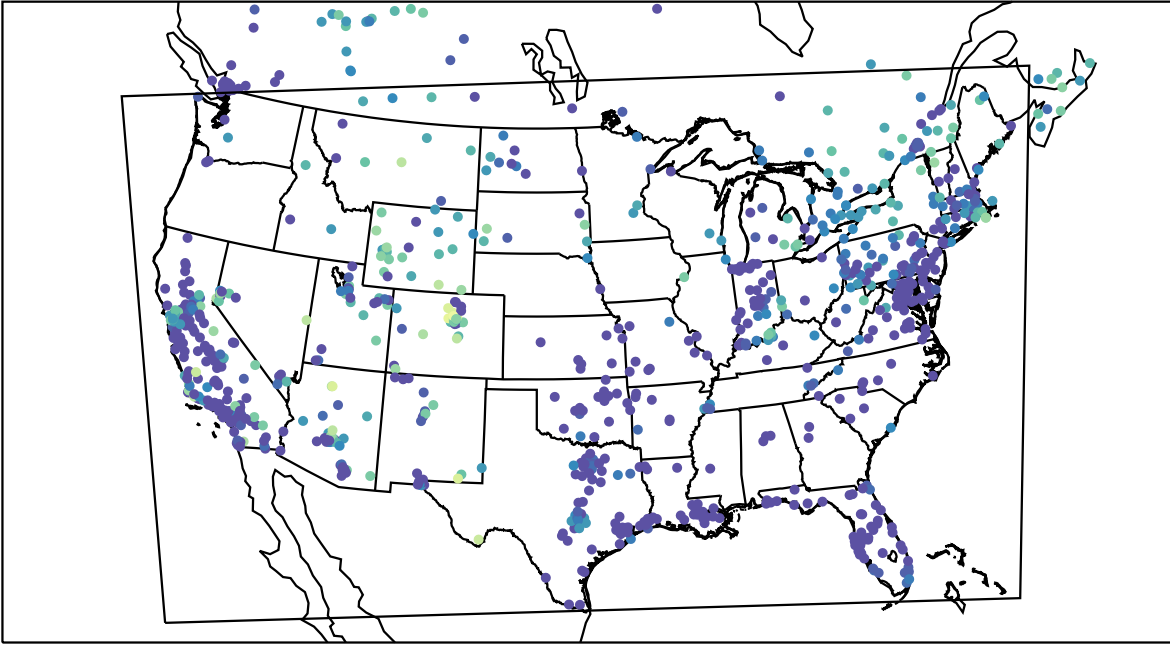
AirNOW (2020-11-11_08:00:00)
