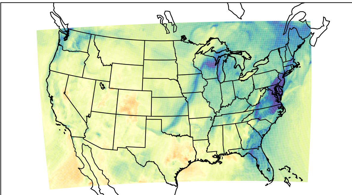
WRF (2020-11-12_20:00:00)
