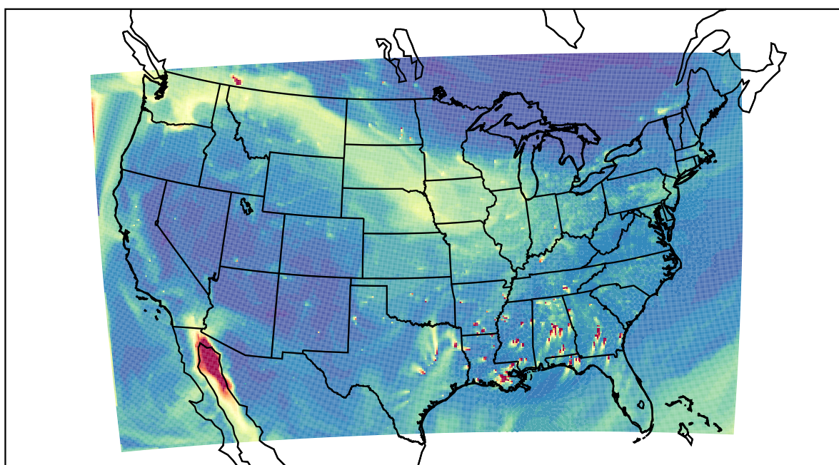
WRF 2020-11-16_22:00:00
