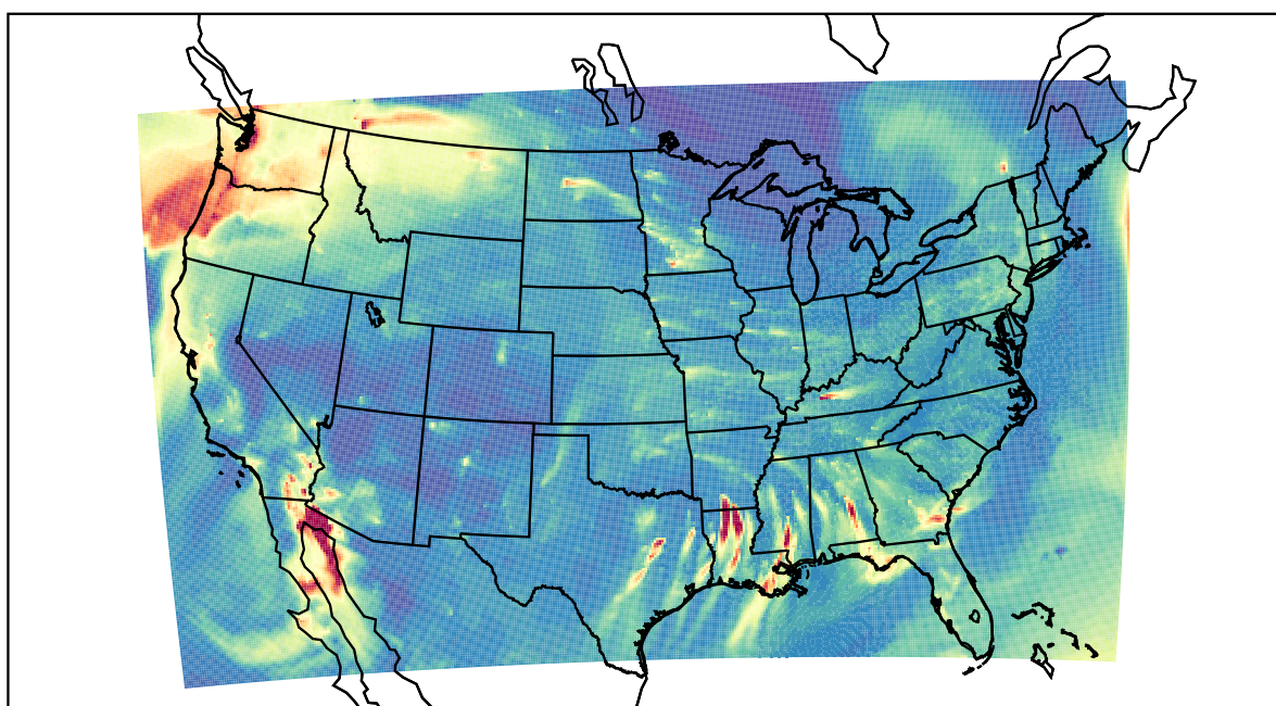
WRF 2020-11-16_04:00:00
