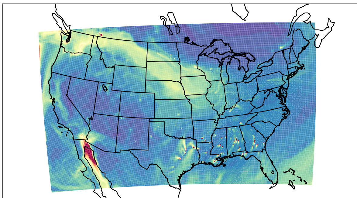
WRF 2020-11-16_20:00:00
