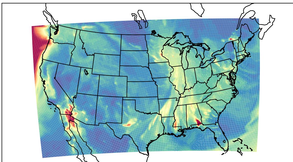
WRF 2020-11-15_06:00:00
