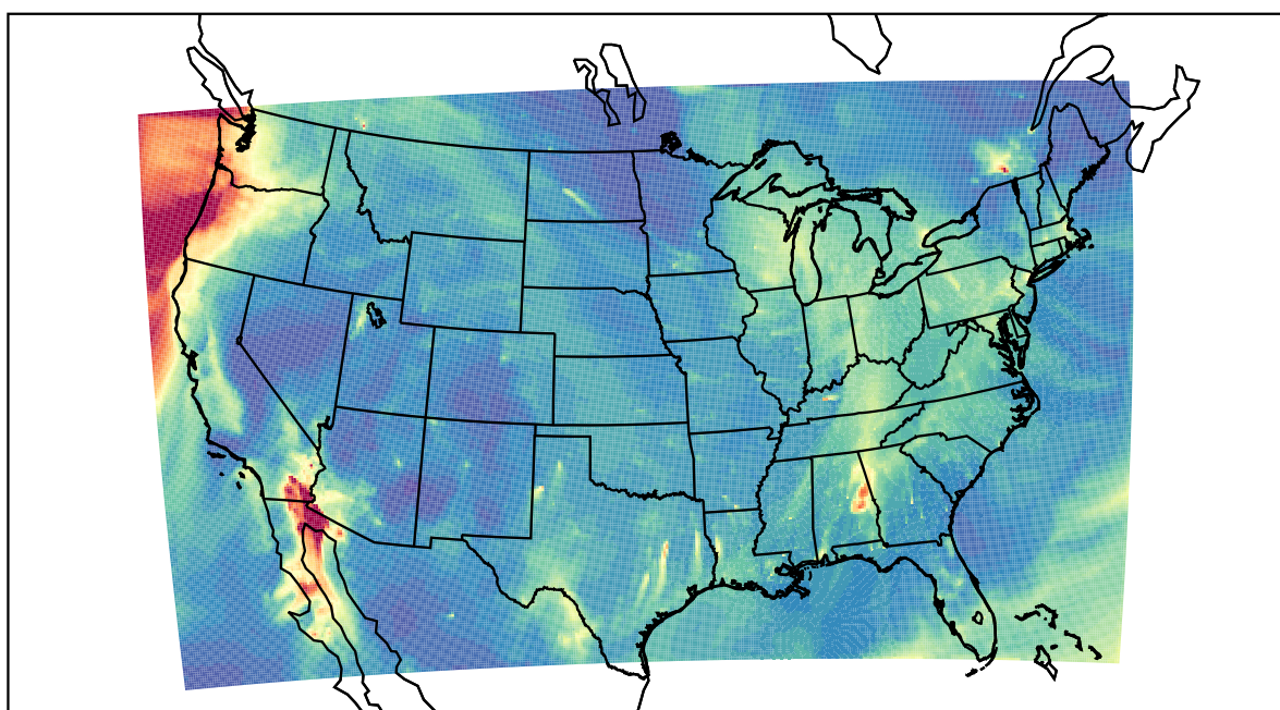
WRF 2020-11-15_13:00:00
