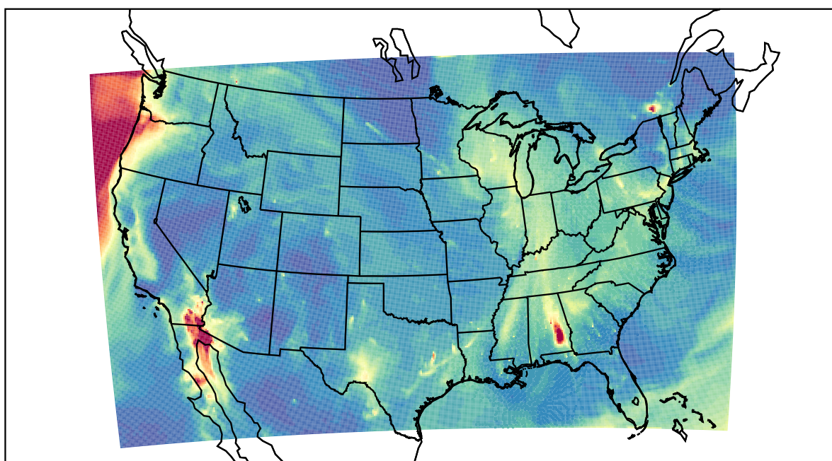
WRF 2020-11-15_10:00:00
