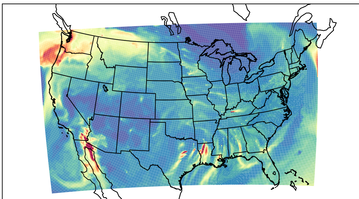
WRF 2020-11-16_07:00:00
