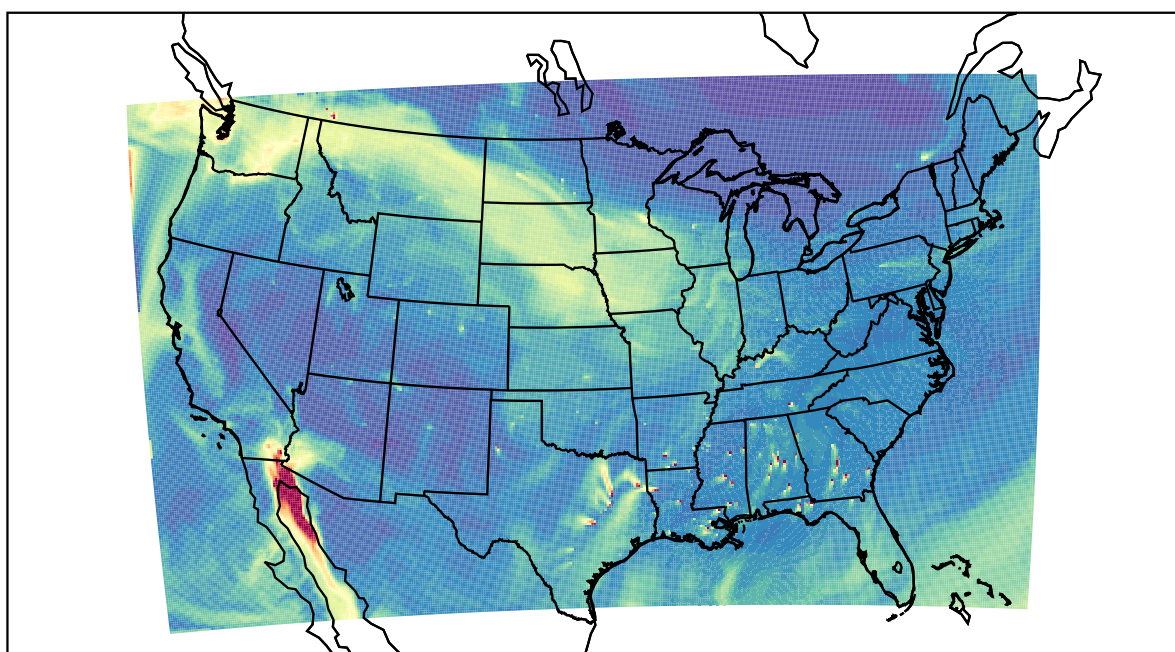
WRF 2020-11-16_19:00:00
