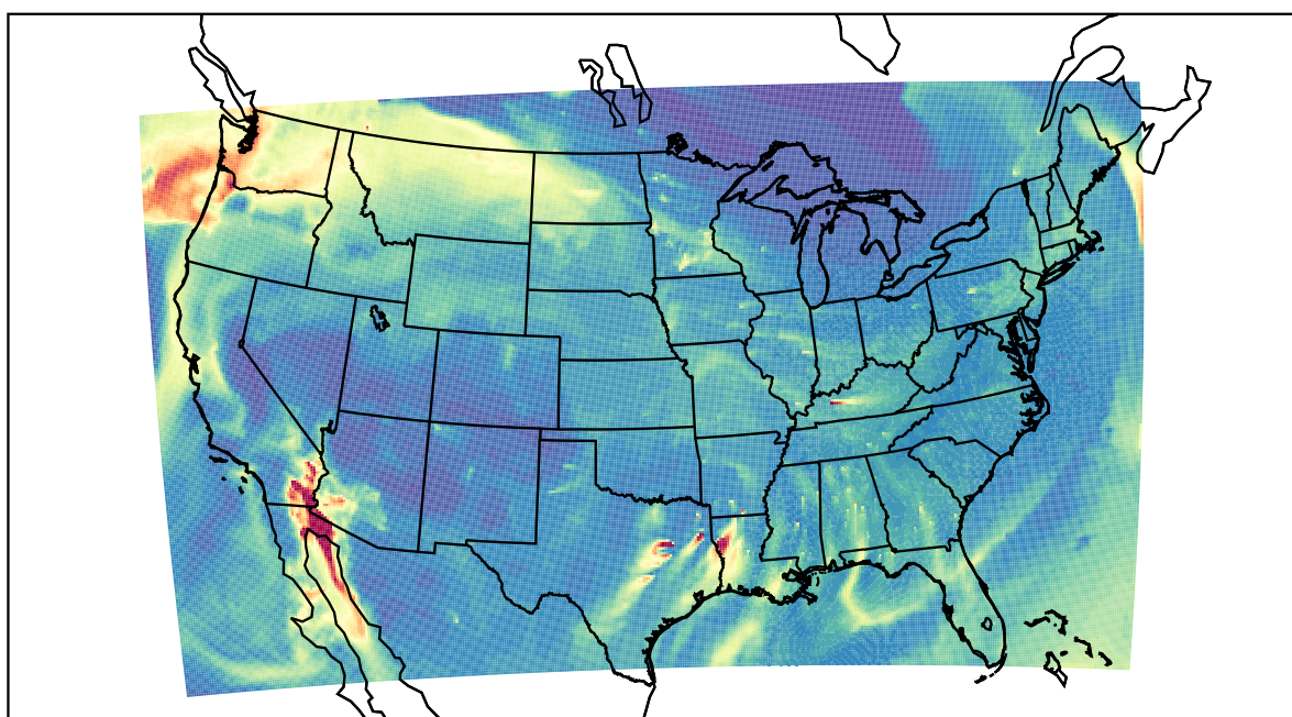
WRF 2020-11-16_10:00:00
