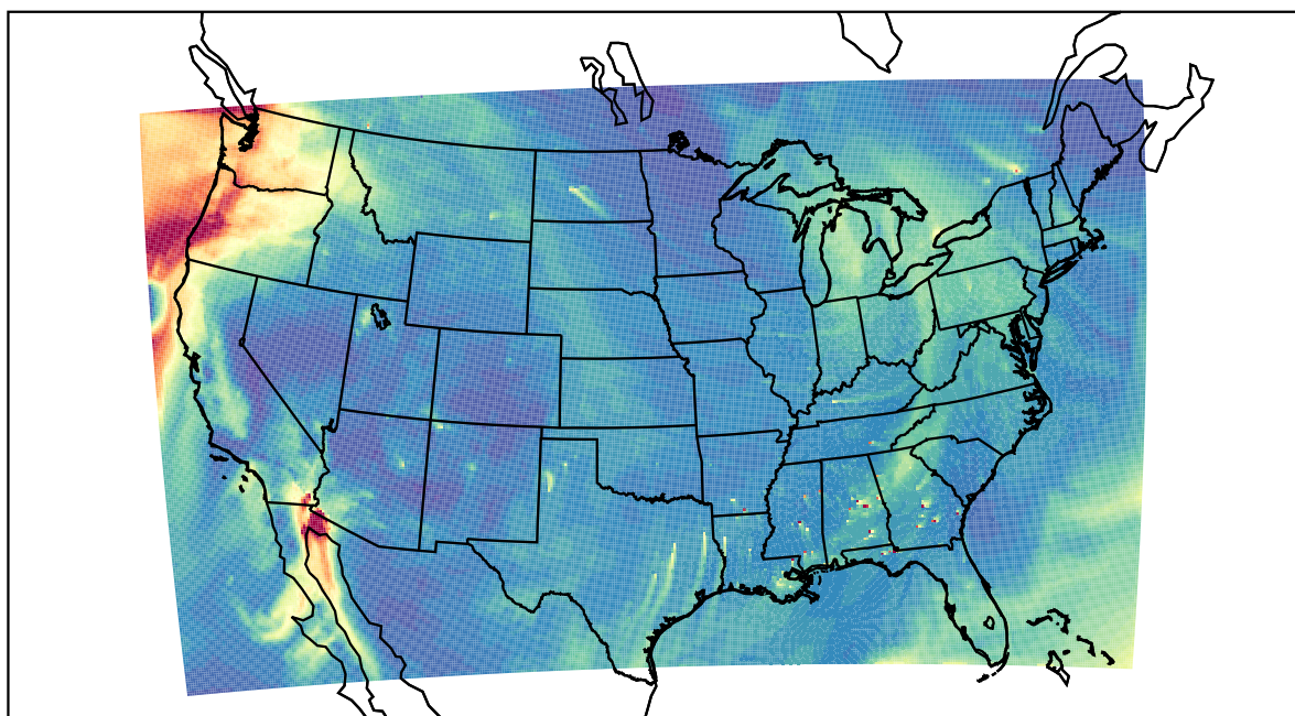
WRF 2020-11-15_18:00:00
