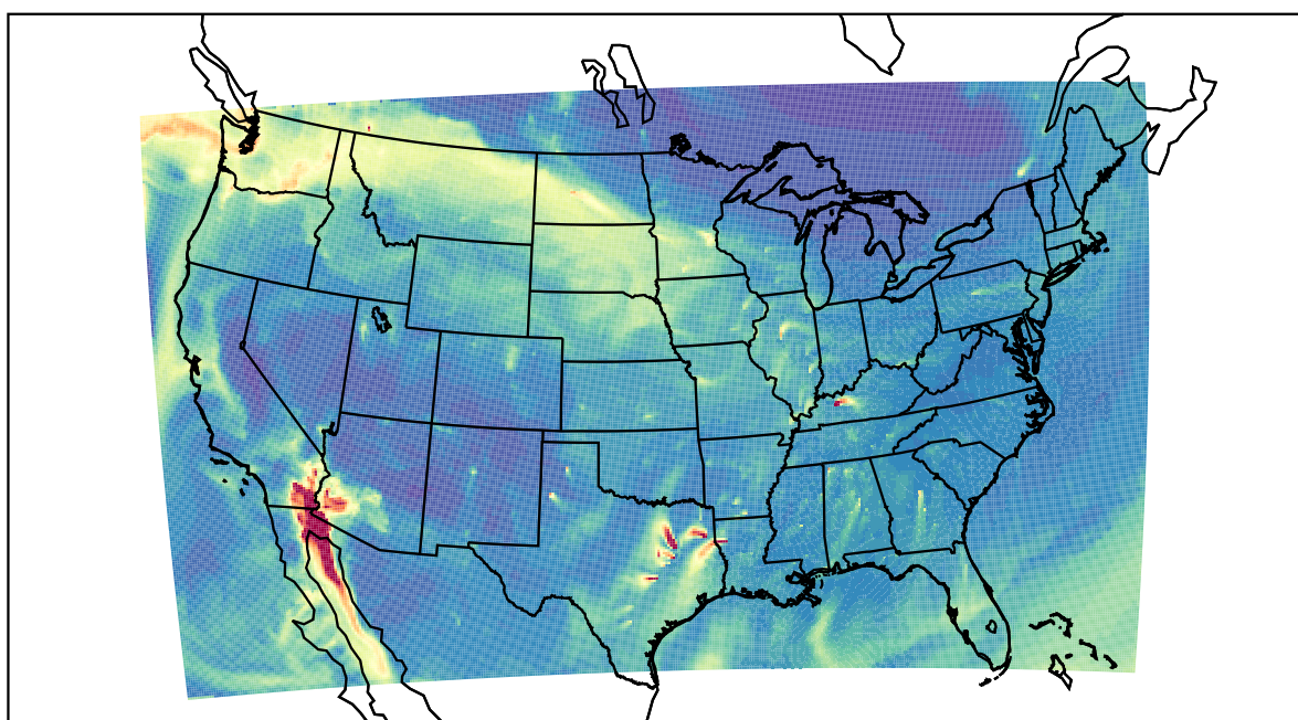
WRF 2020-11-16_16:00:00
