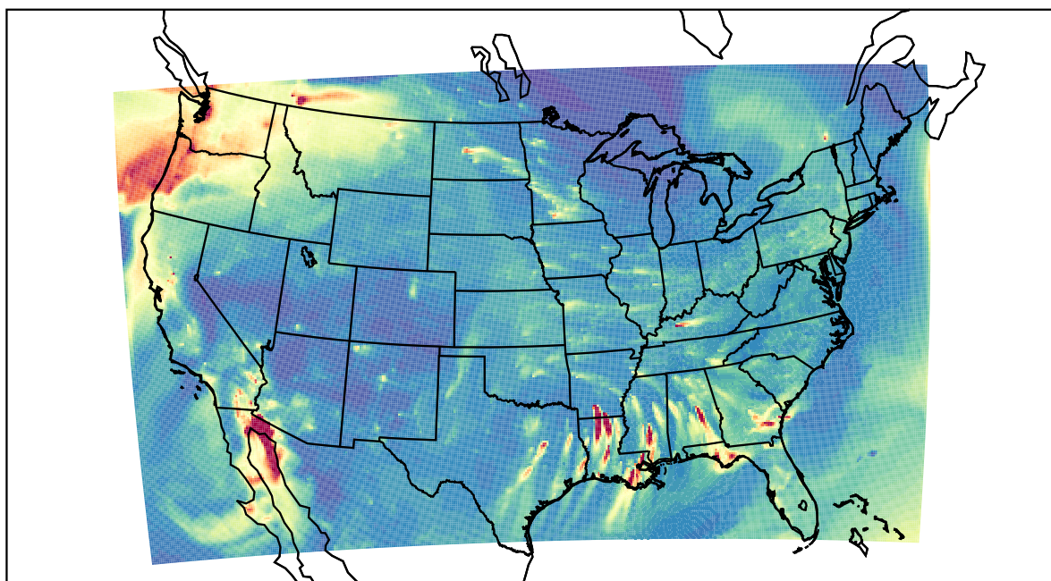
WRF 2020-11-16_03:00:00
