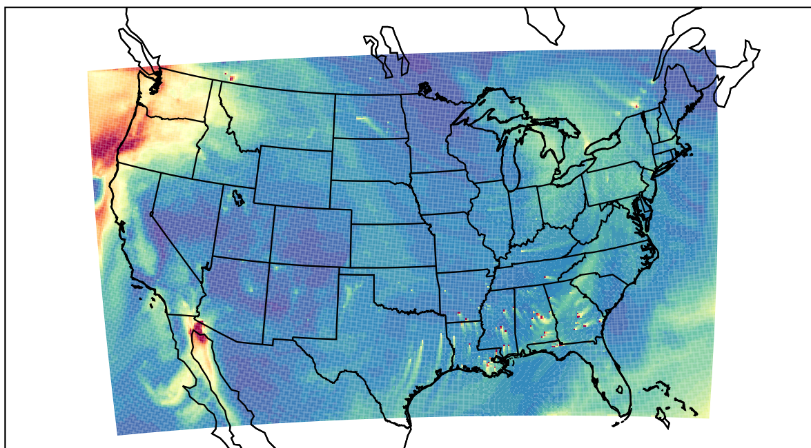
WRF 2020-11-15_20:00:00
