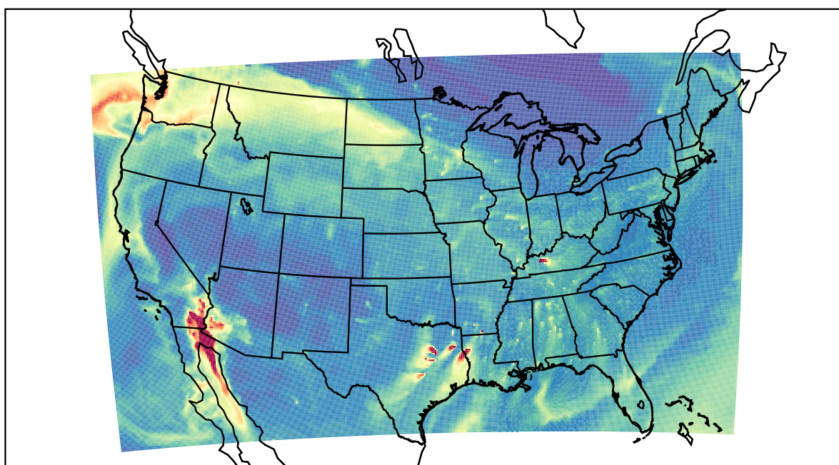
WRF 2020-11-16_13:00:00
