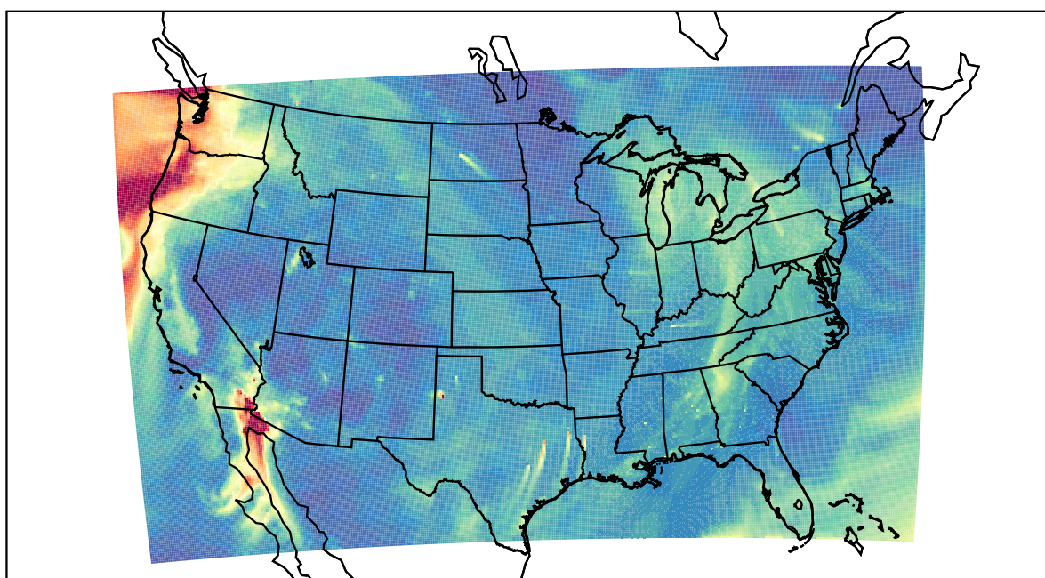
WRF 2020-11-15_16:00:00
