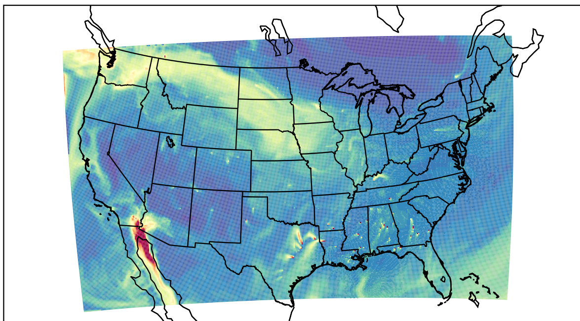
WRF 2020-11-16_18:00:00
