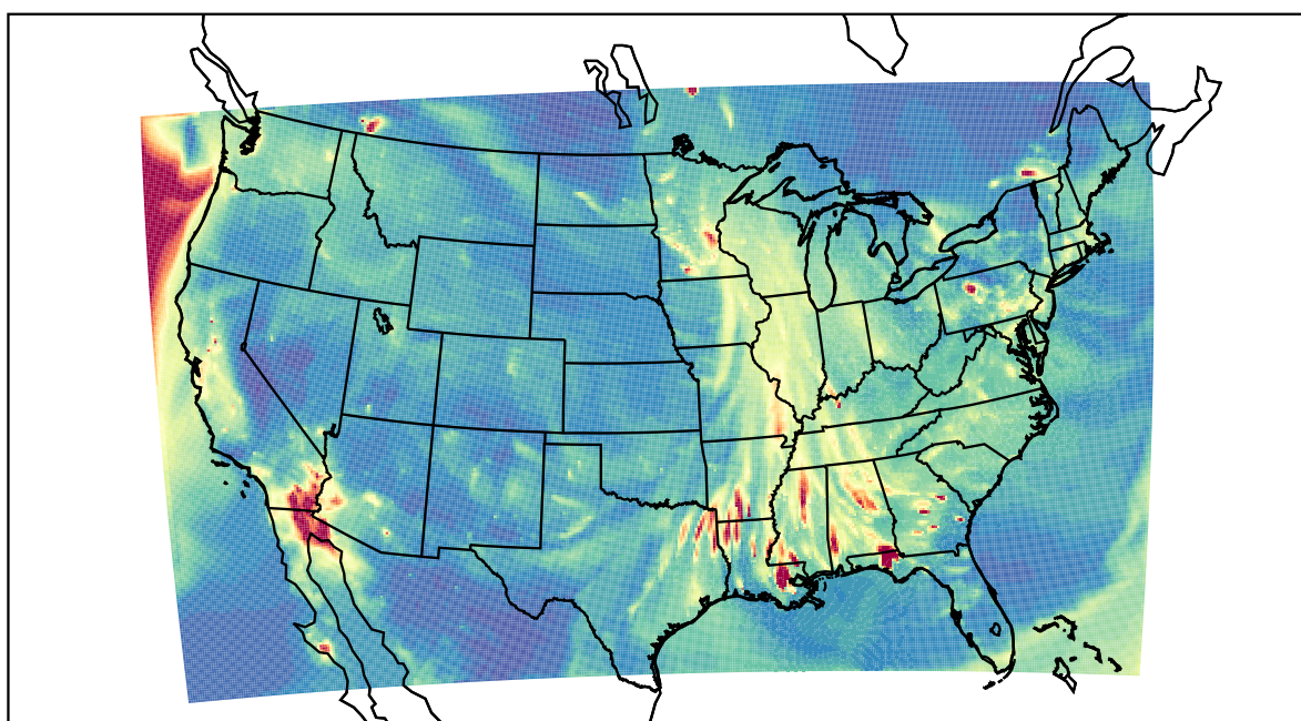
WRF 2020-11-15_03:00:00
