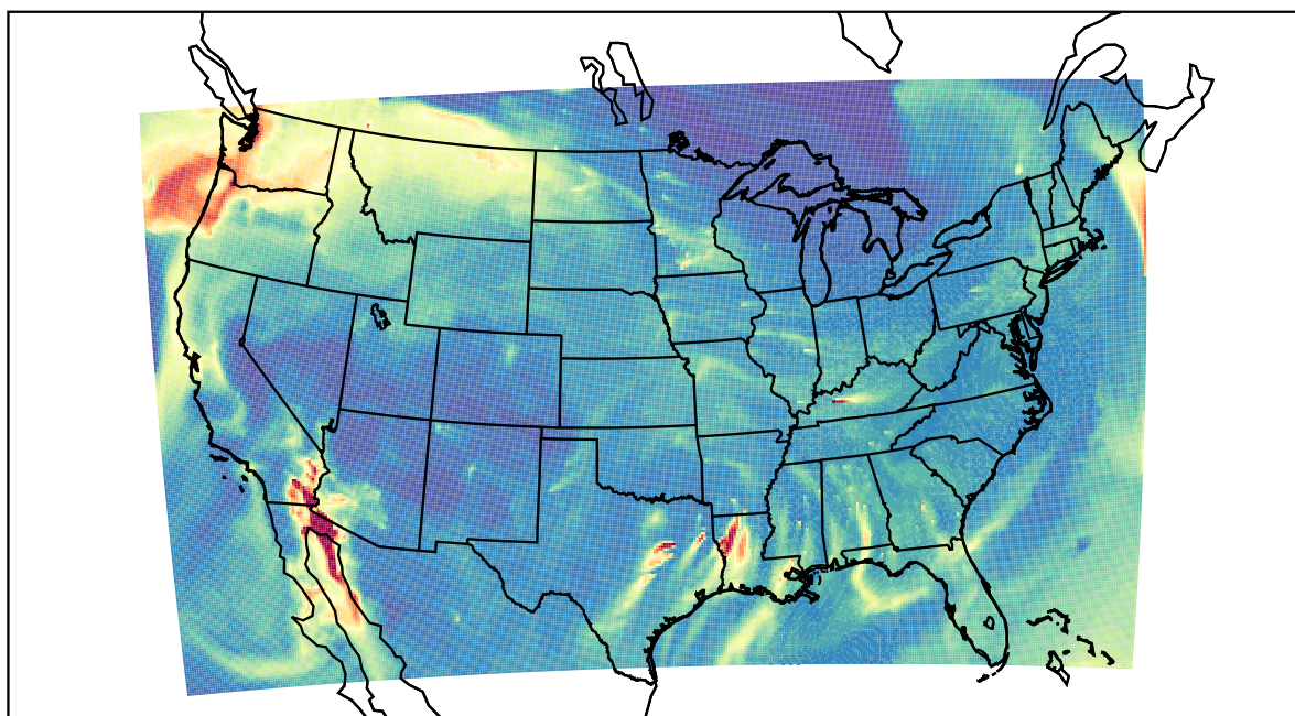
WRF 2020-11-16_08:00:00
