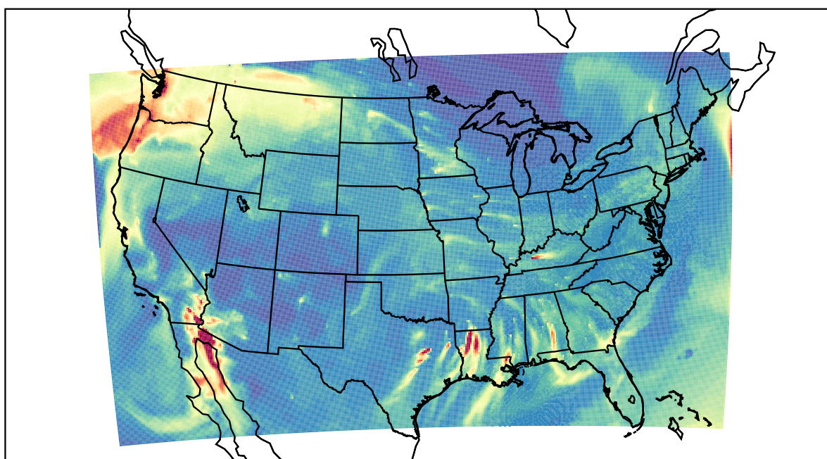
WRF 2020-11-16_06:00:00
