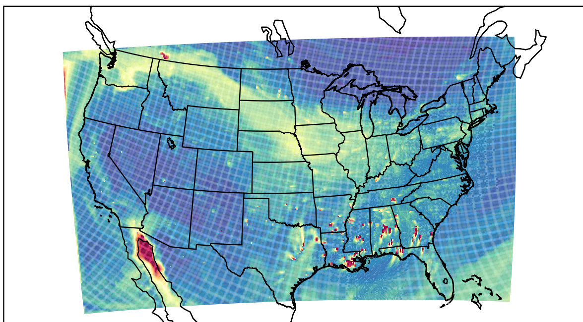
WRF 2020-11-16_23:00:00
