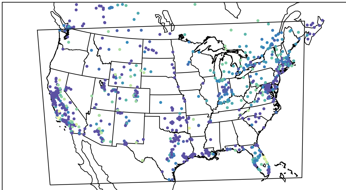
AirNOW (2020-11-17_08:00:00)
