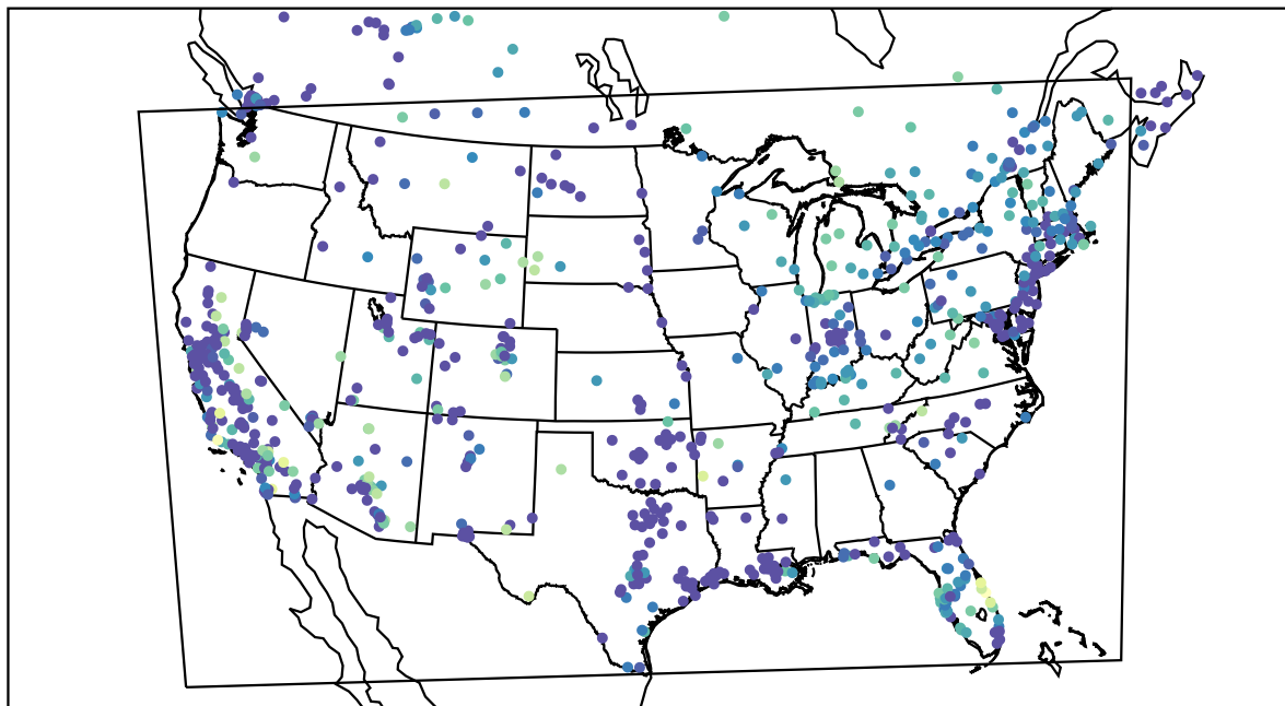
AirNOW (2020-11-17_09:00:00)
