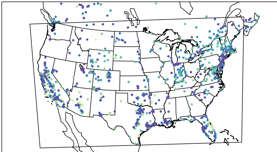
AirNOW (2020-11-17_01:00:00)
