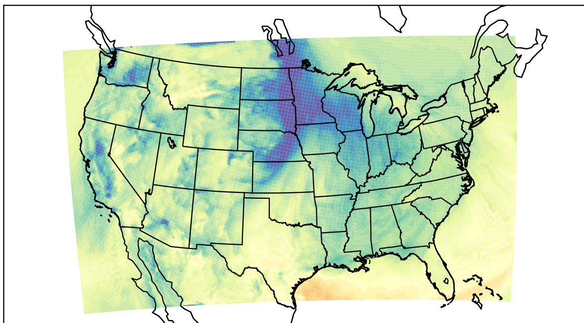
WRF (2020-11-18_18:00:00)
