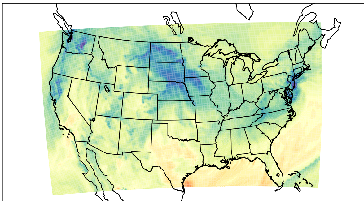
WRF (2020-11-17_20:00:00)
