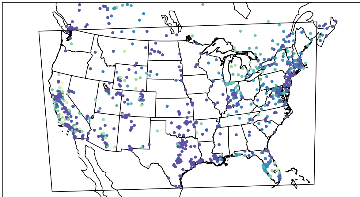
AirNOW (2020-11-17_13:00:00)
