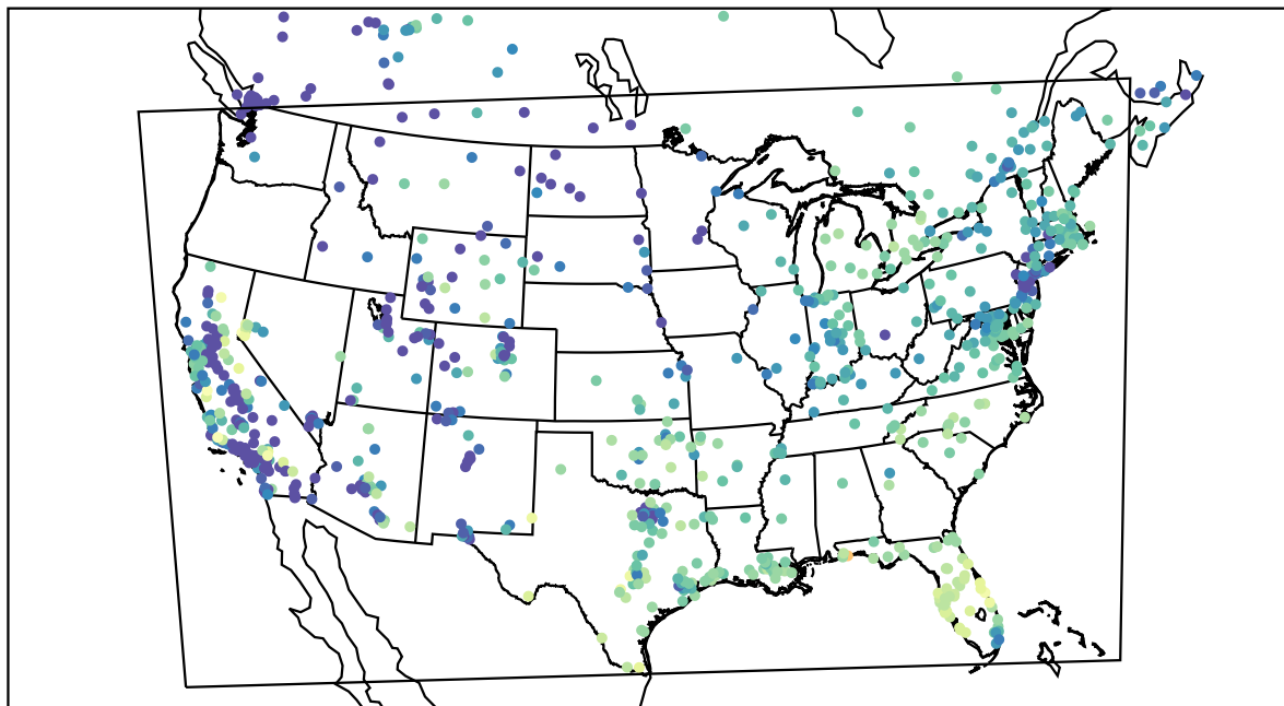
AirNOW (2020-11-17_16:00:00)
