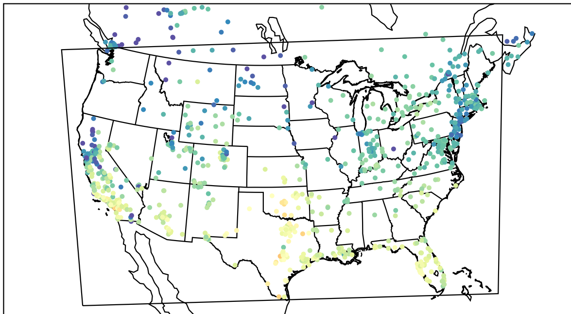
AirNOW (2020-11-17_20:00:00)
