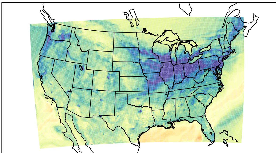
WRF (2020-11-17_00:00:00)
