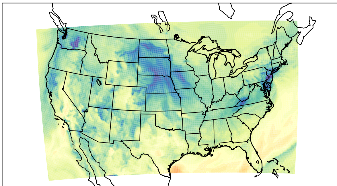
WRF (2020-11-17_18:00:00)
