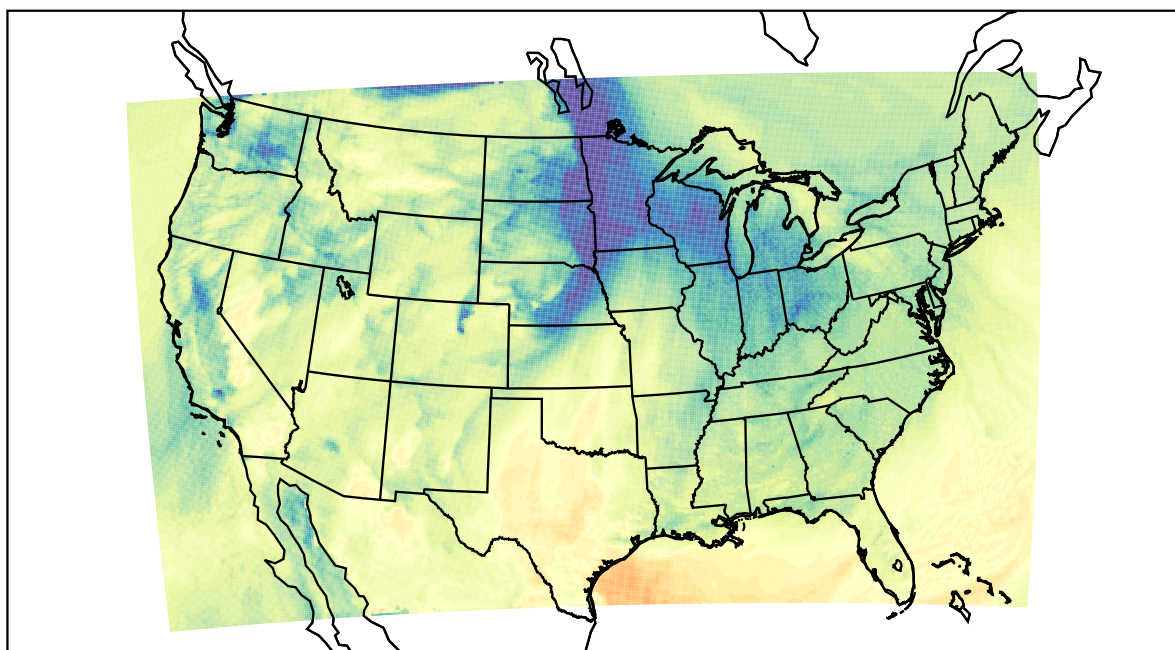
WRF (2020-11-18_20:00:00)
