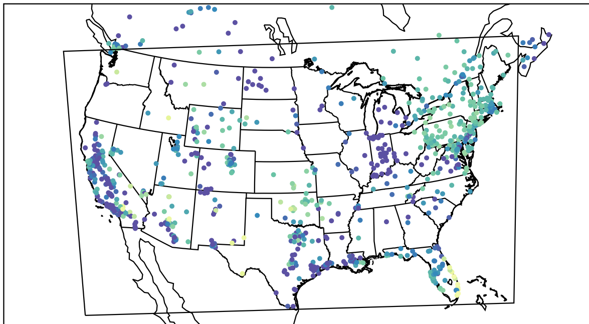
AirNOW (2020-11-18_10:00:00)
