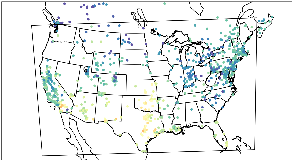
AirNOW (2020-11-18_22:00:00)
