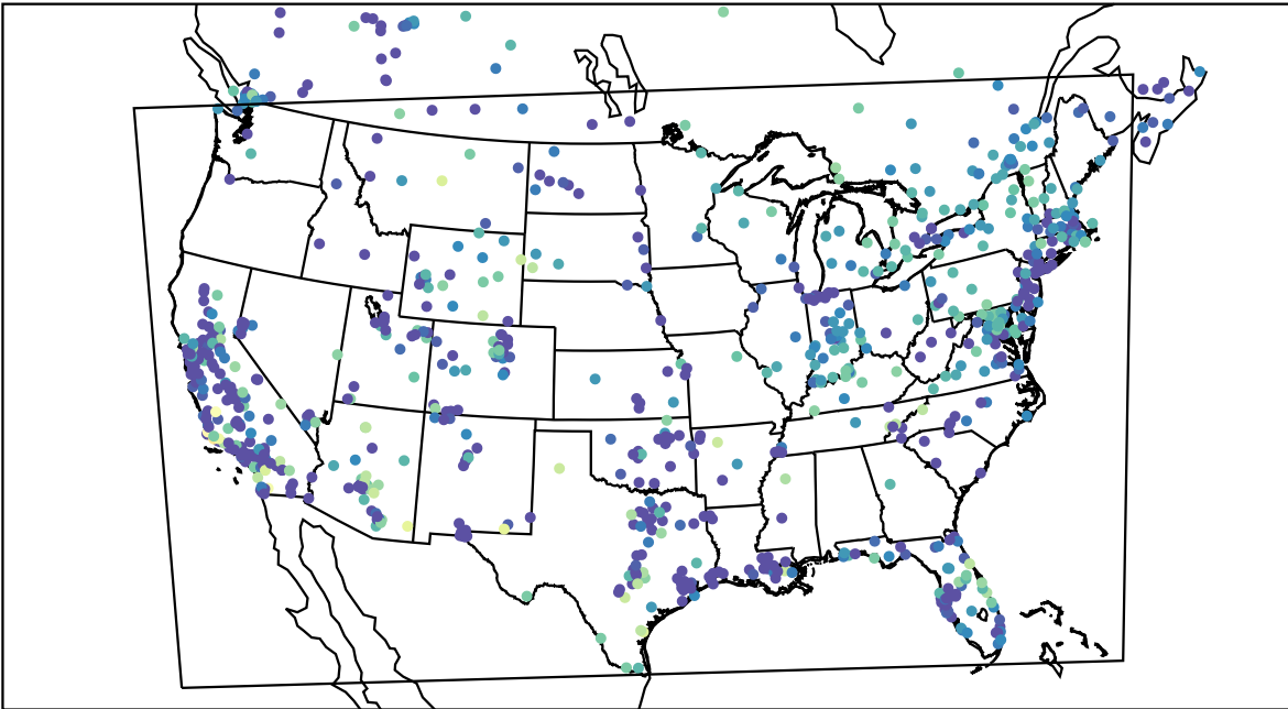
AirNOW (2020-11-17_03:00:00)
