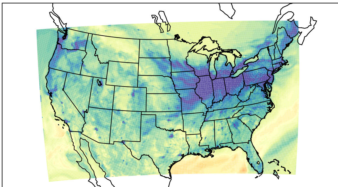
WRF (2020-11-17_01:00:00)
