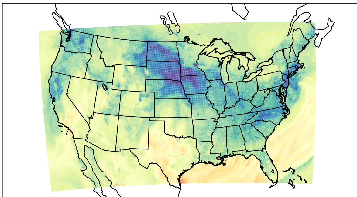
WRF (2020-11-17_22:00:00)
