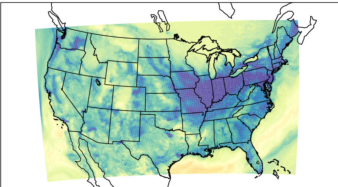
WRF (2020-11-17_06:00:00)
