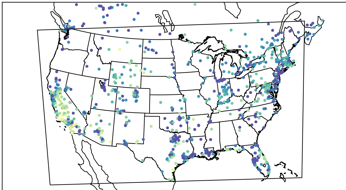
AirNOW (2020-11-17_00:00:00)
