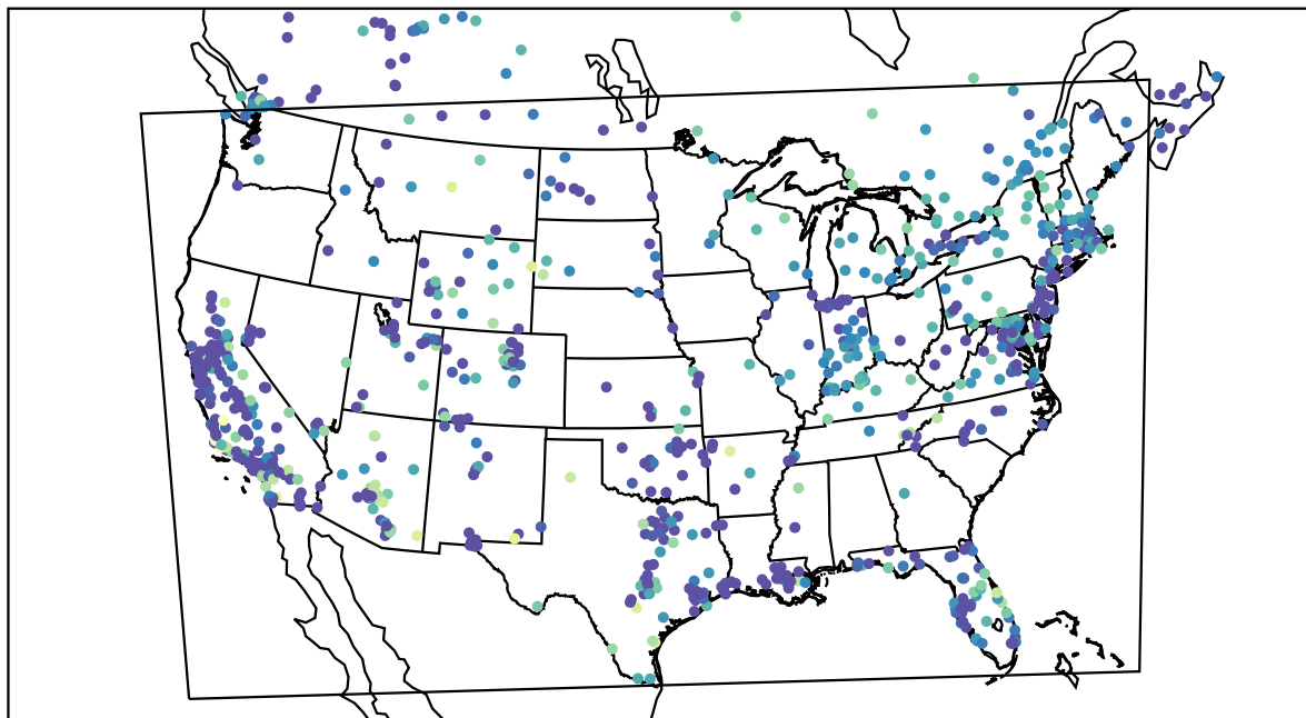
AirNOW (2020-11-17_04:00:00)
