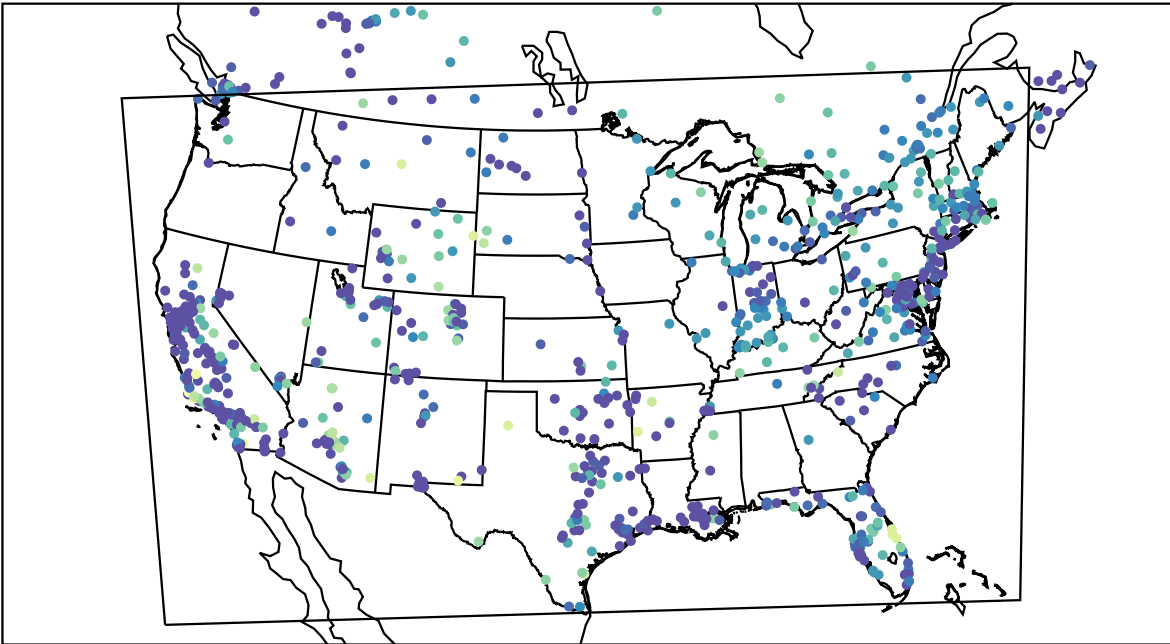
AirNOW (2020-11-17_06:00:00)
