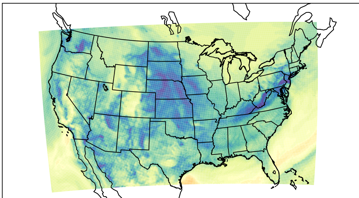
WRF (2020-11-17_16:00:00)
