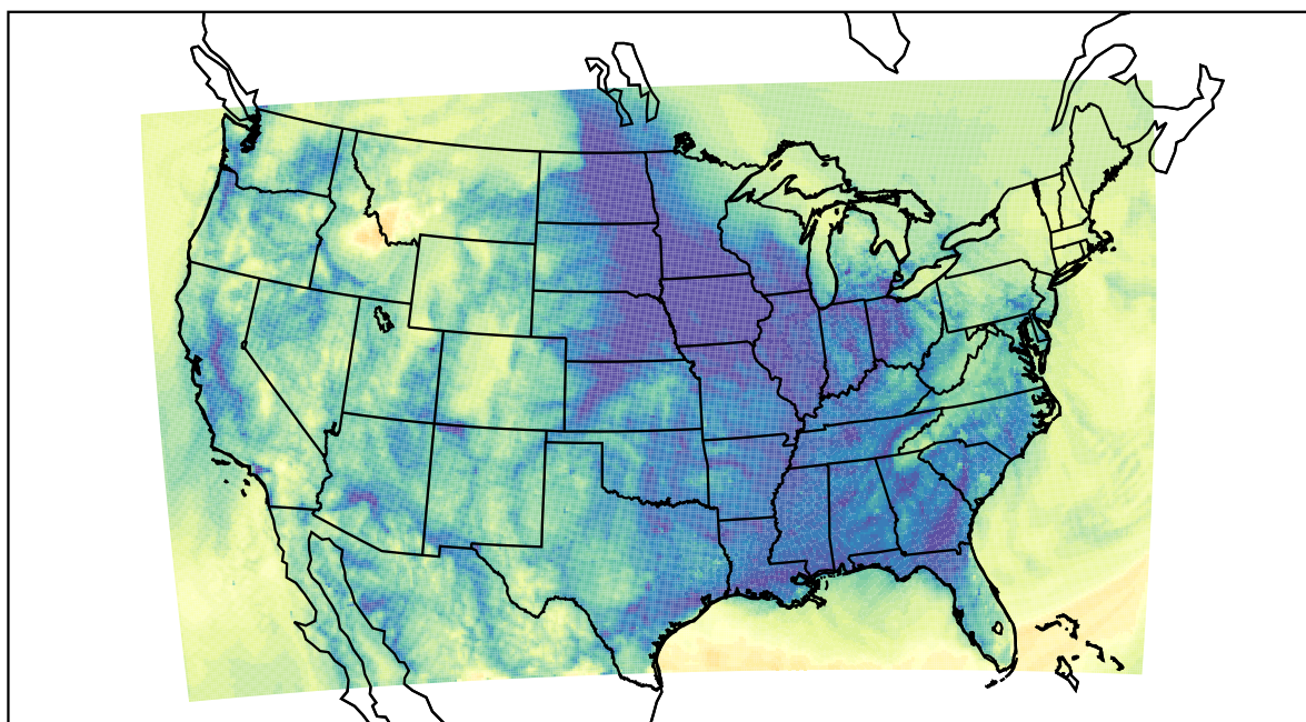
WRF (2020-11-18_13:00:00)
