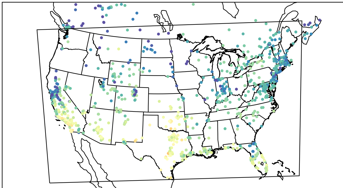
AirNOW (2020-11-17_22:00:00)
