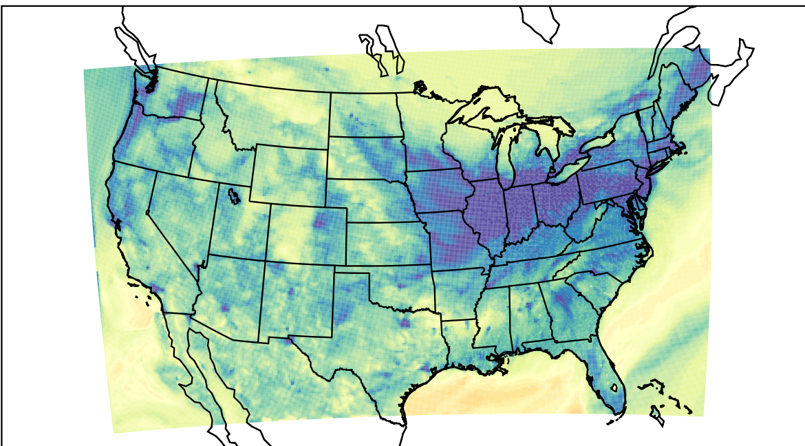
WRF (2020-11-17_03:00:00)
