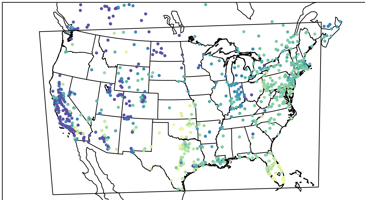
AirNOW (2020-11-18_16:00:00)
