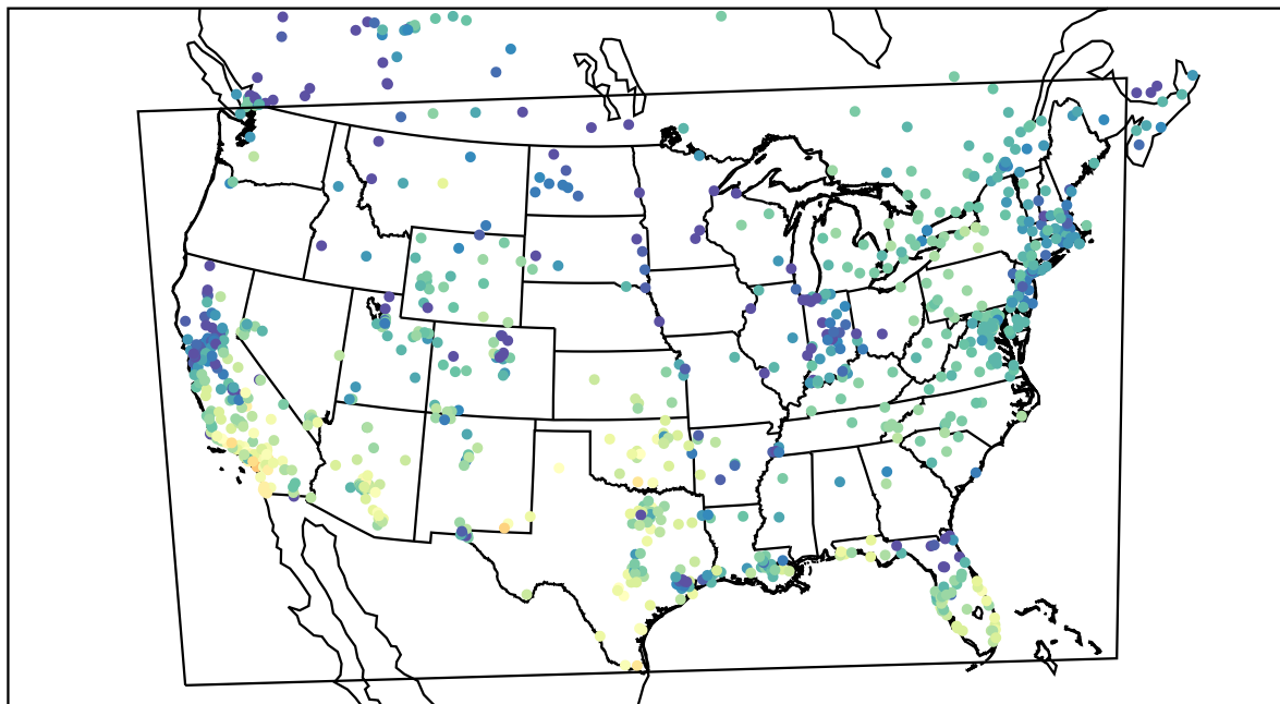
AirNOW (2020-11-17_23:00:00)
