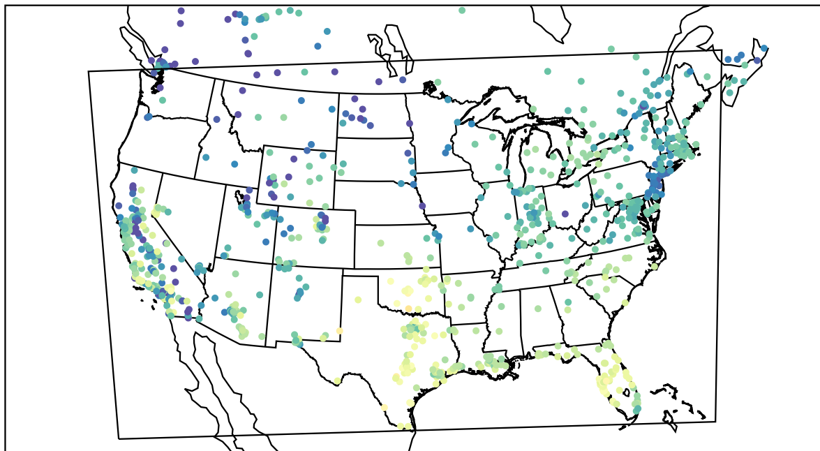
AirNOW (2020-11-17_18:00:00)
