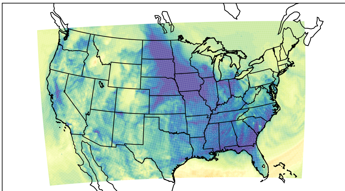
WRF (2020-11-18_10:00:00)
