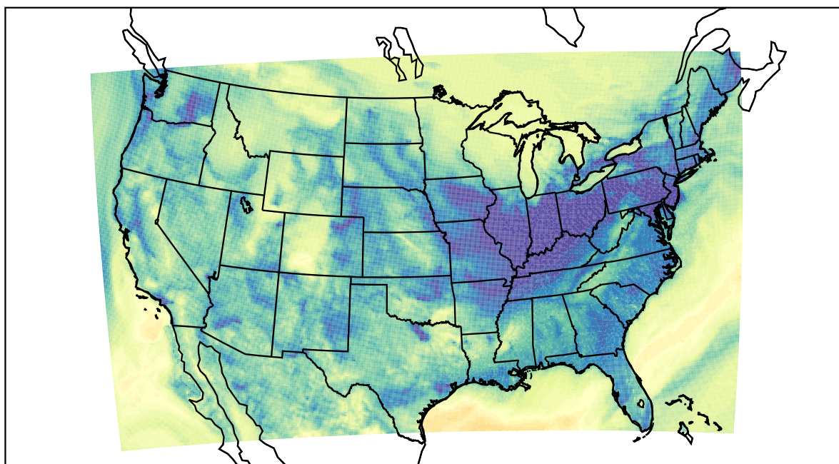
WRF (2020-11-17_08:00:00)
