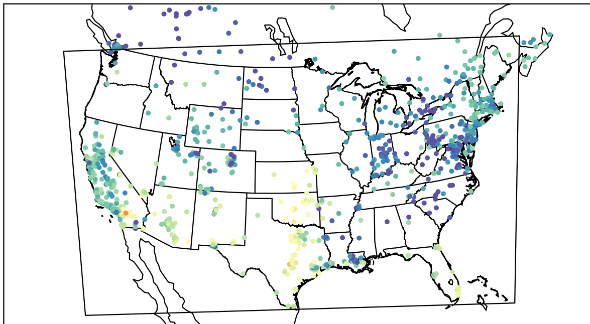
AirNOW (2020-11-18_23:00:00)
