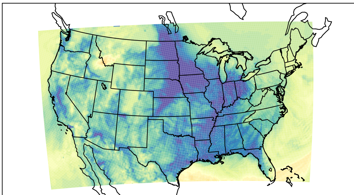
WRF (2020-11-18_14:00:00)
