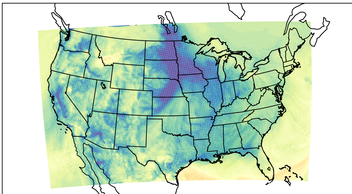
WRF (2020-11-18_16:00:00)
