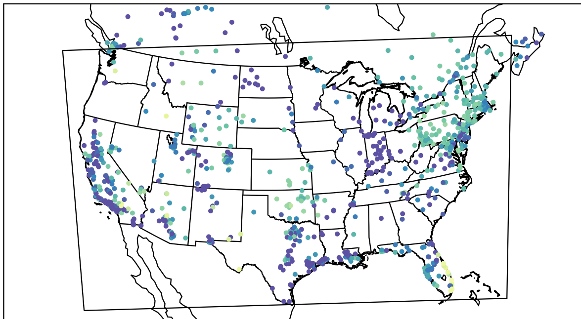
AirNOW (2020-11-18_11:00:00)
