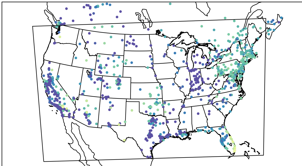
AirNOW (2020-11-18_13:00:00)
