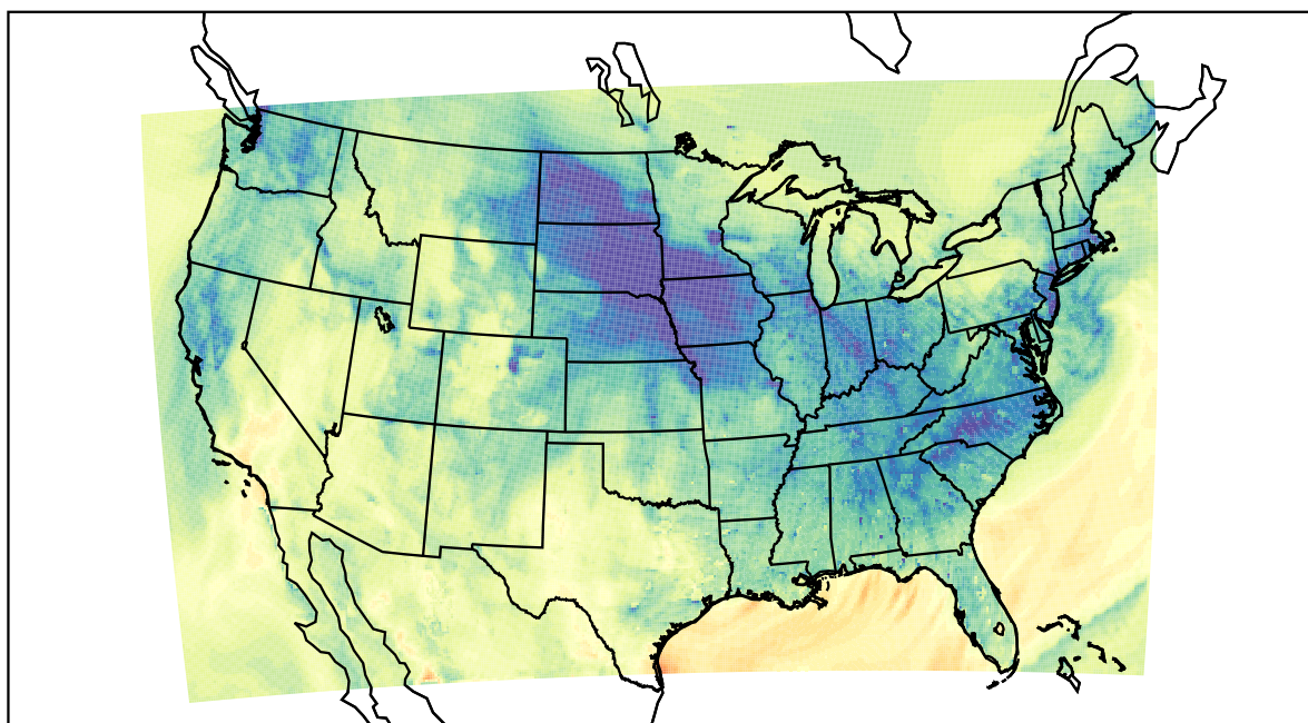
WRF (2020-11-17_23:00:00)
