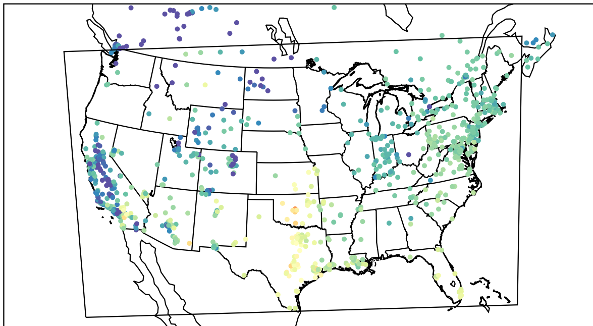
AirNOW (2020-11-18_18:00:00)
