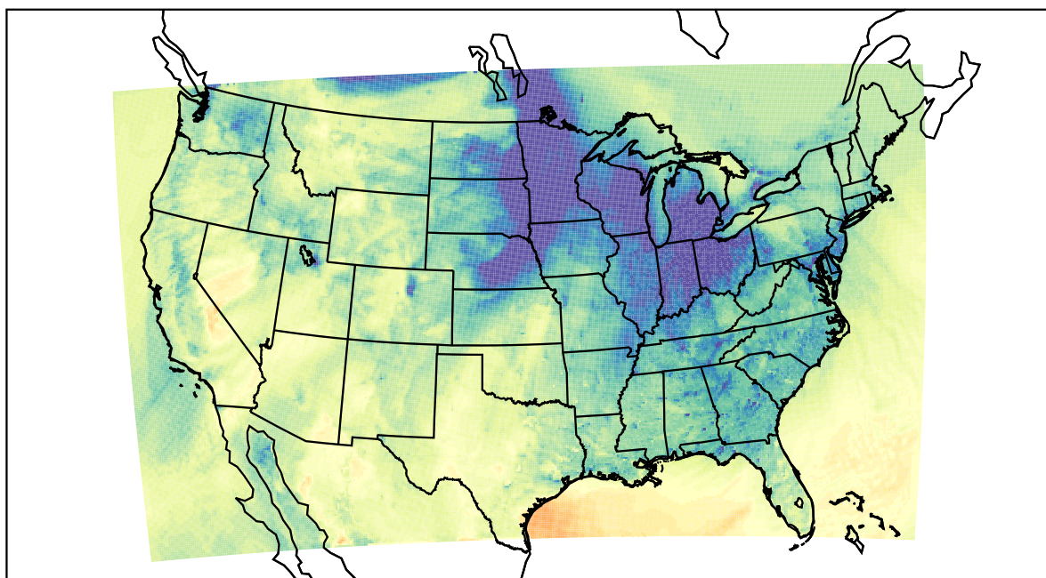
WRF (2020-11-18_23:00:00)
