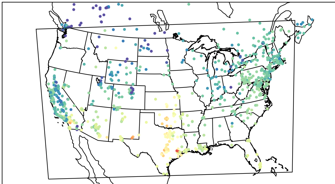
AirNOW (2020-11-18_20:00:00)
