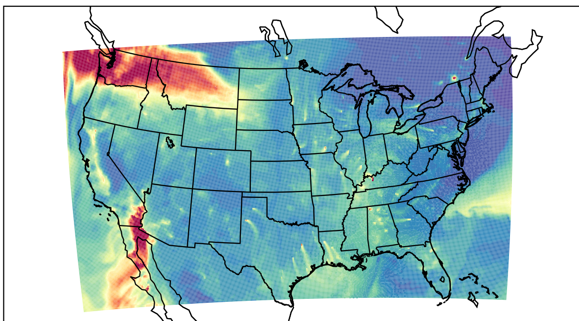
WRF 2020-12-16_16:00:00
