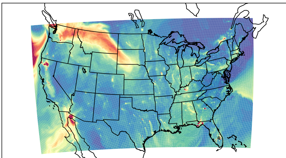
WRF 2020-12-16_23:00:00
