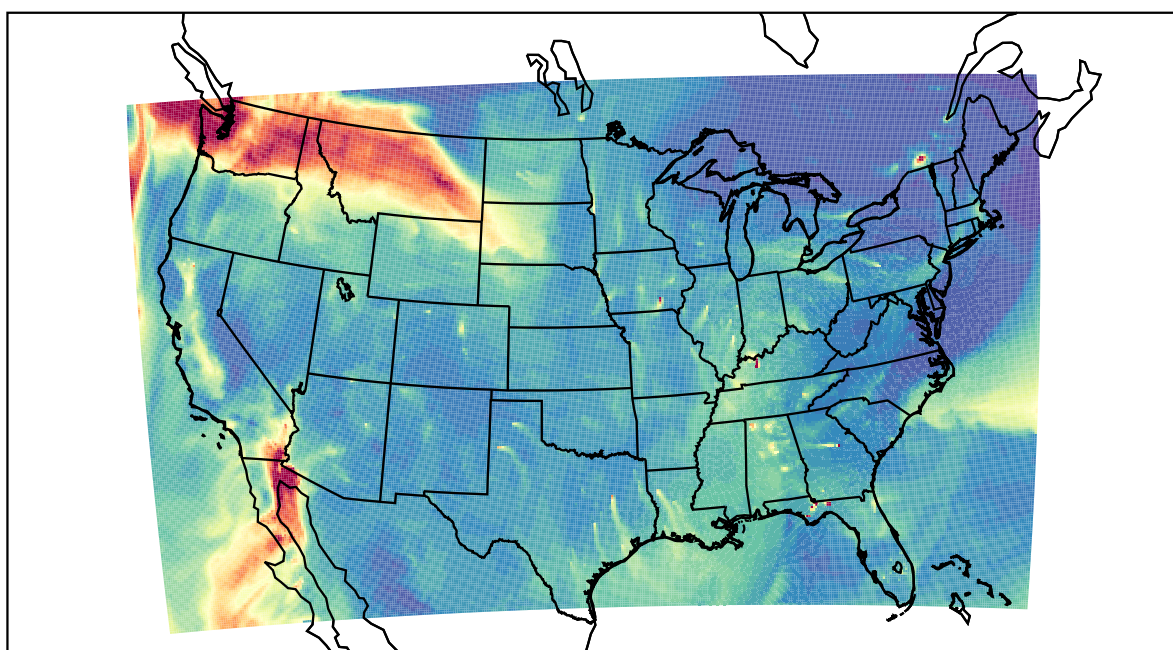
WRF 2020-12-16_18:00:00
