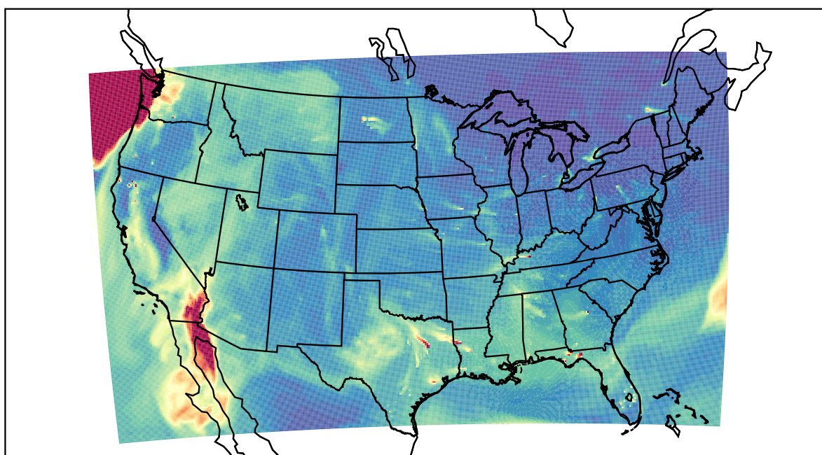
WRF 2020-12-15_20:00:00
