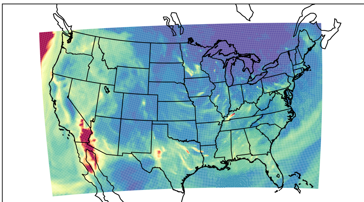
WRF 2020-12-15_10:00:00
