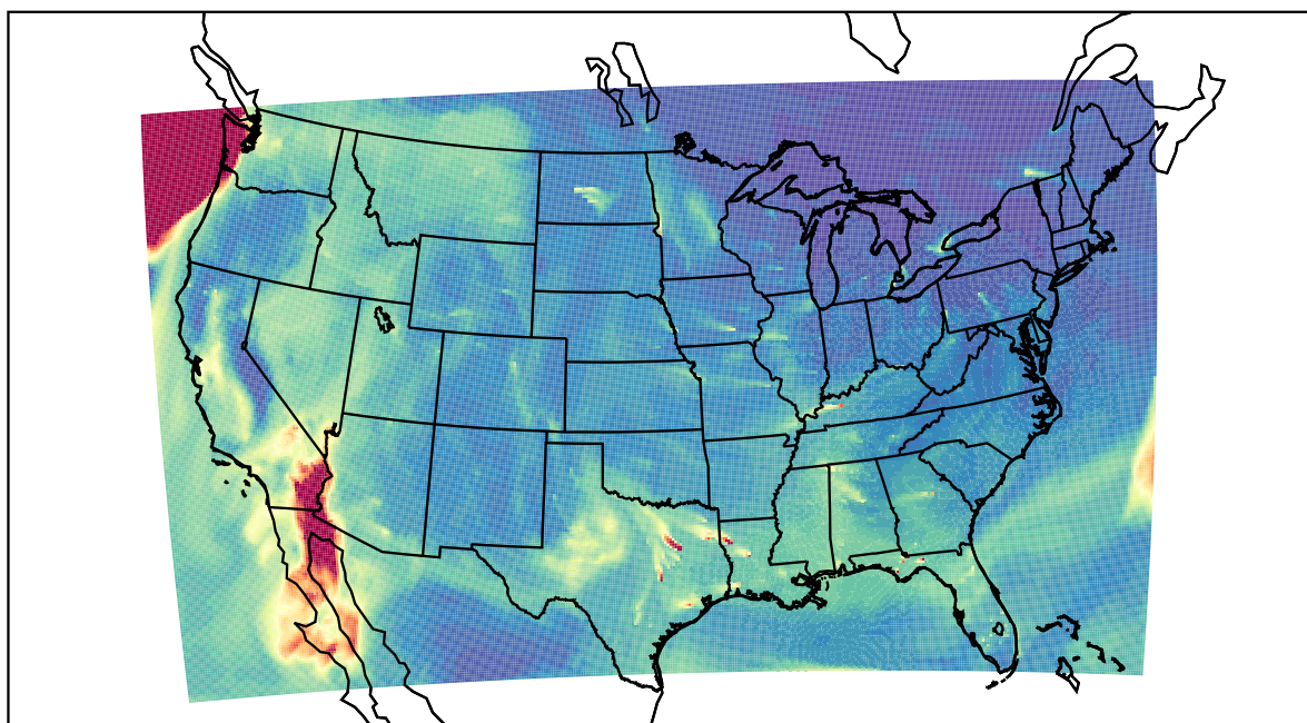
WRF 2020-12-15_18:00:00
