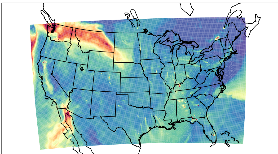
WRF 2020-12-16_20:00:00
