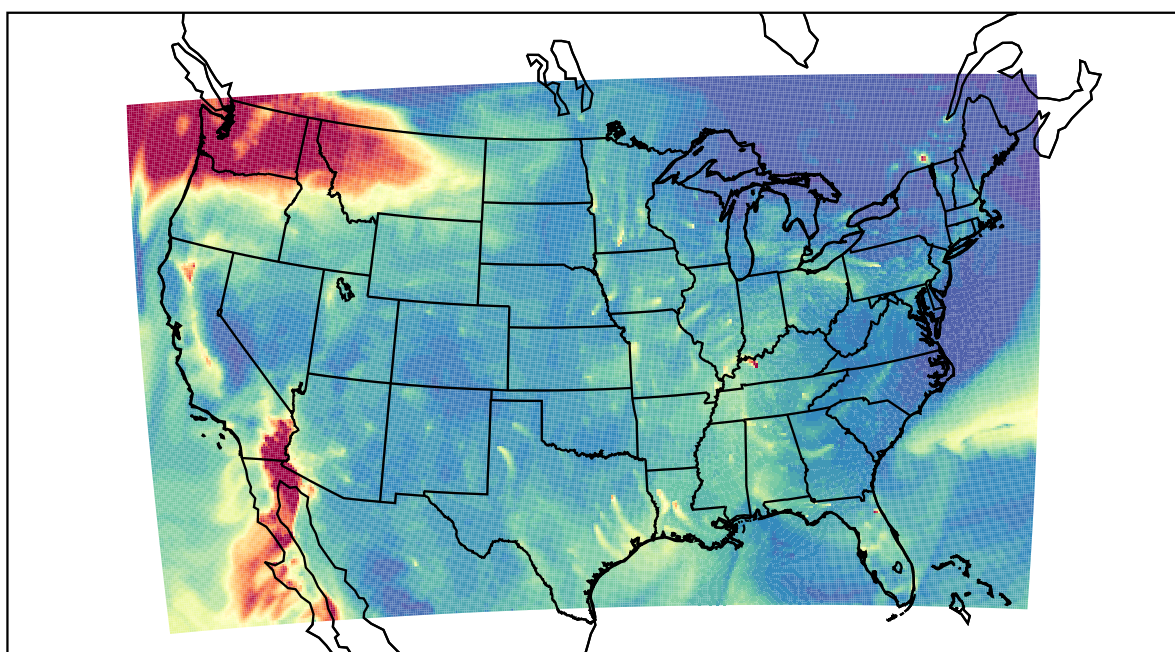
WRF 2020-12-16_13:00:00
