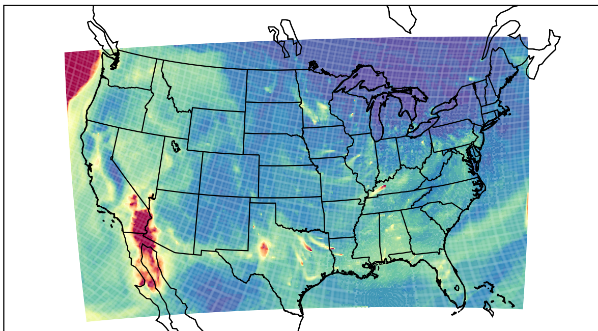
WRF 2020-12-15_13:00:00
