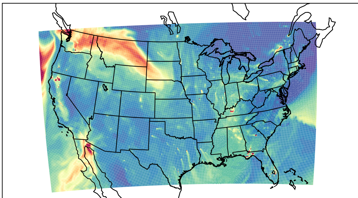
WRF 2020-12-16_22:00:00
