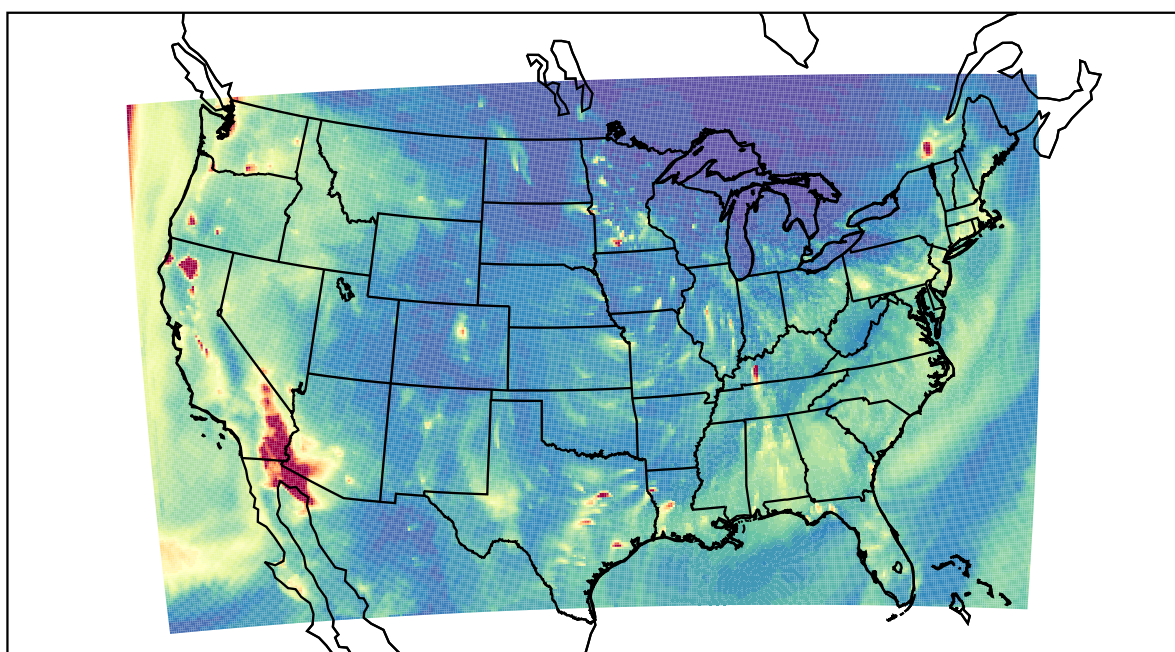
WRF 2020-12-15_03:00:00
