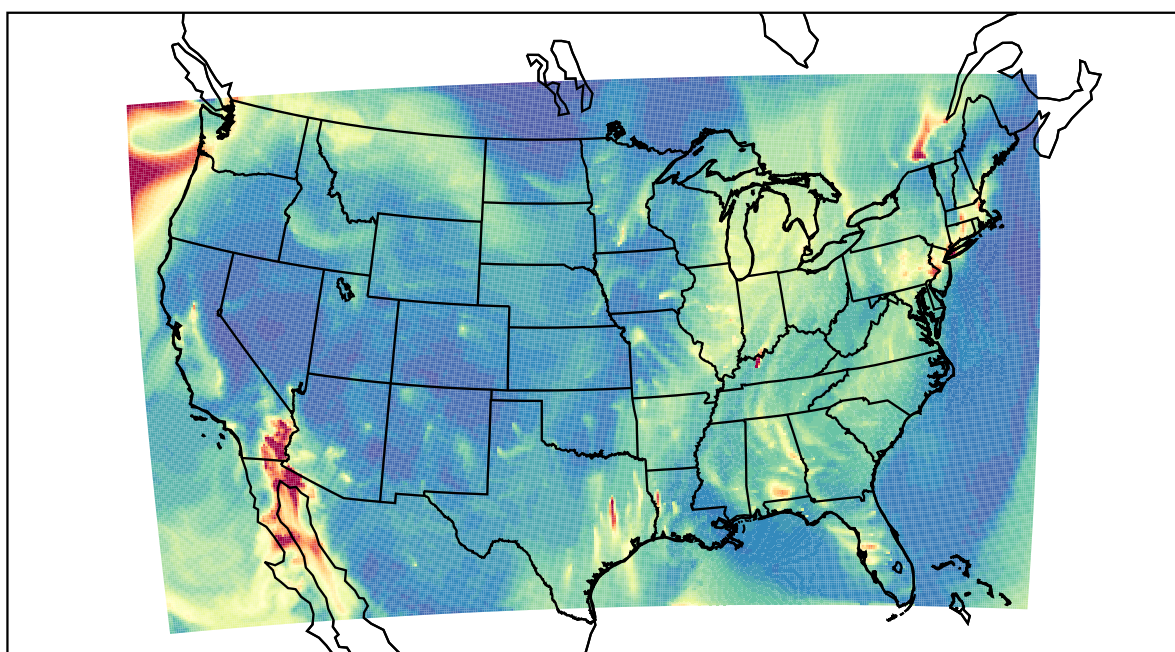
WRF 2020-12-20_06:00:00
