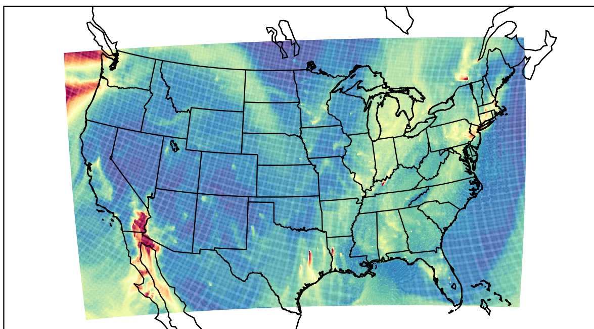
WRF 2020-12-20_10:00:00
