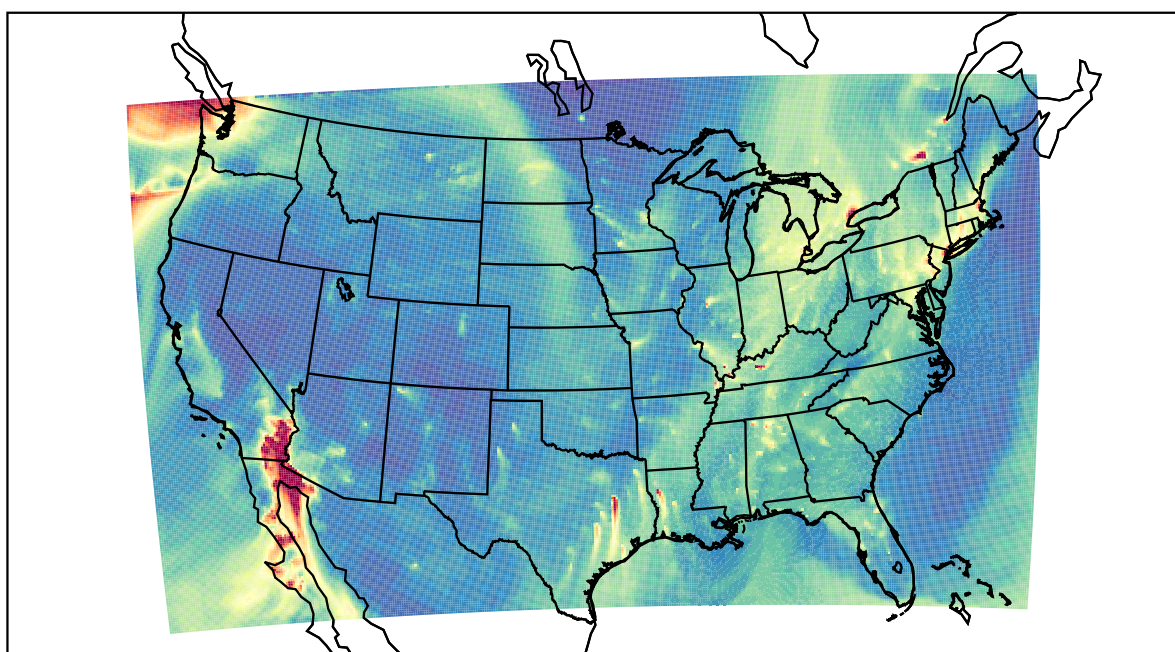
WRF 2020-12-20_15:00:00
