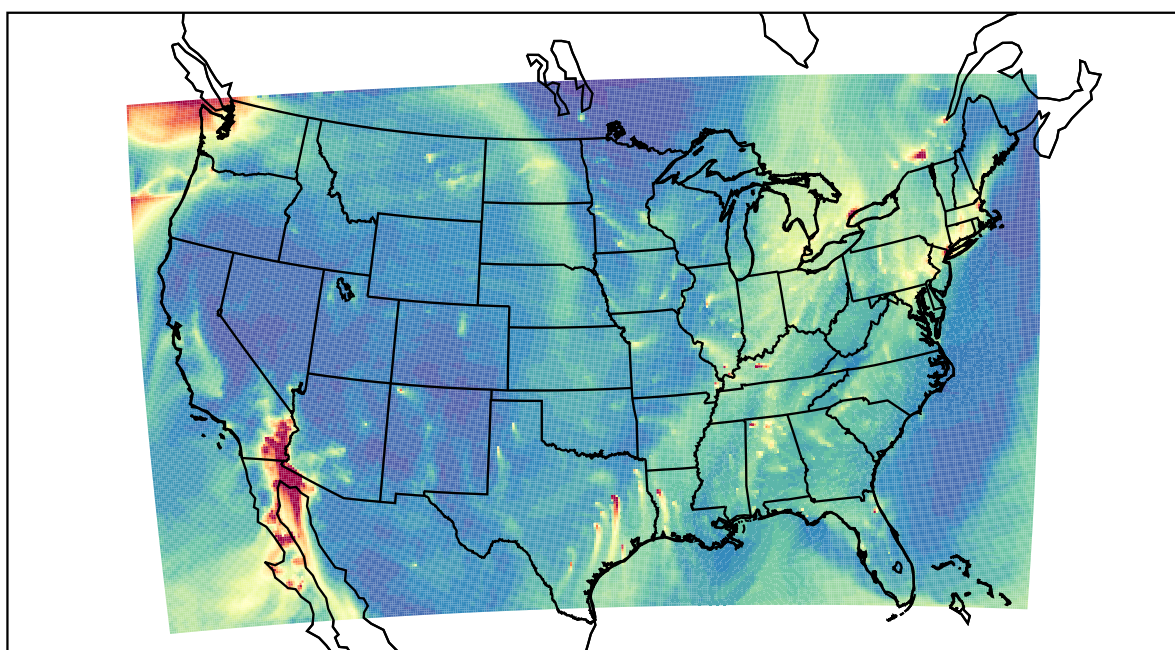
WRF 2020-12-20_16:00:00
