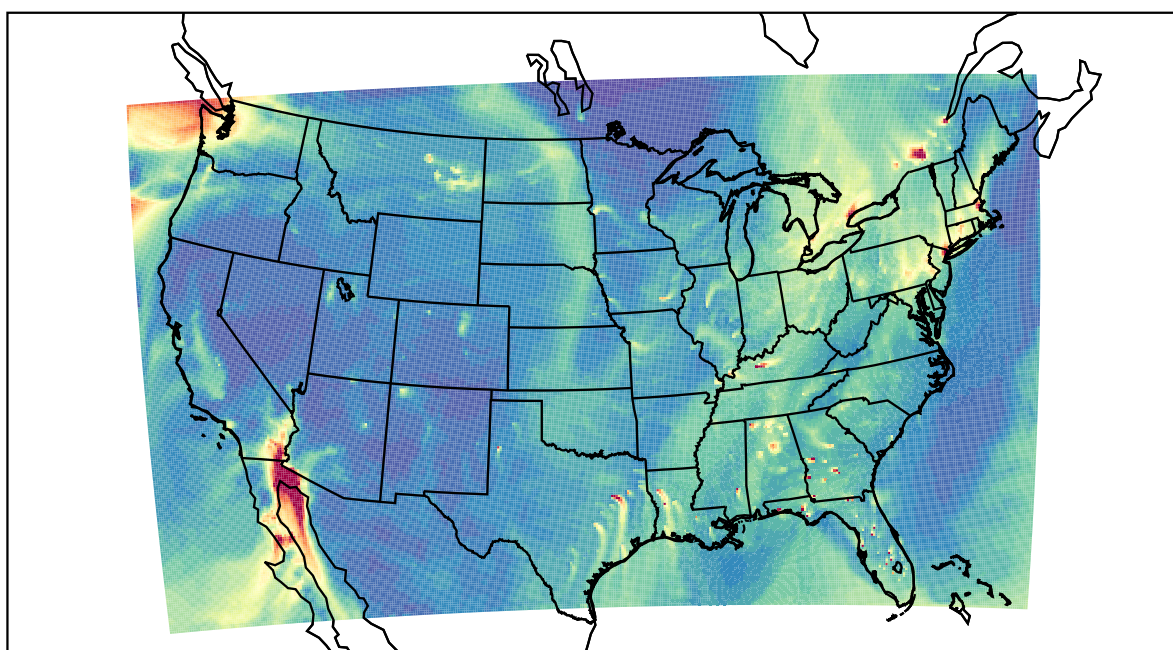
WRF 2020-12-20_19:00:00
