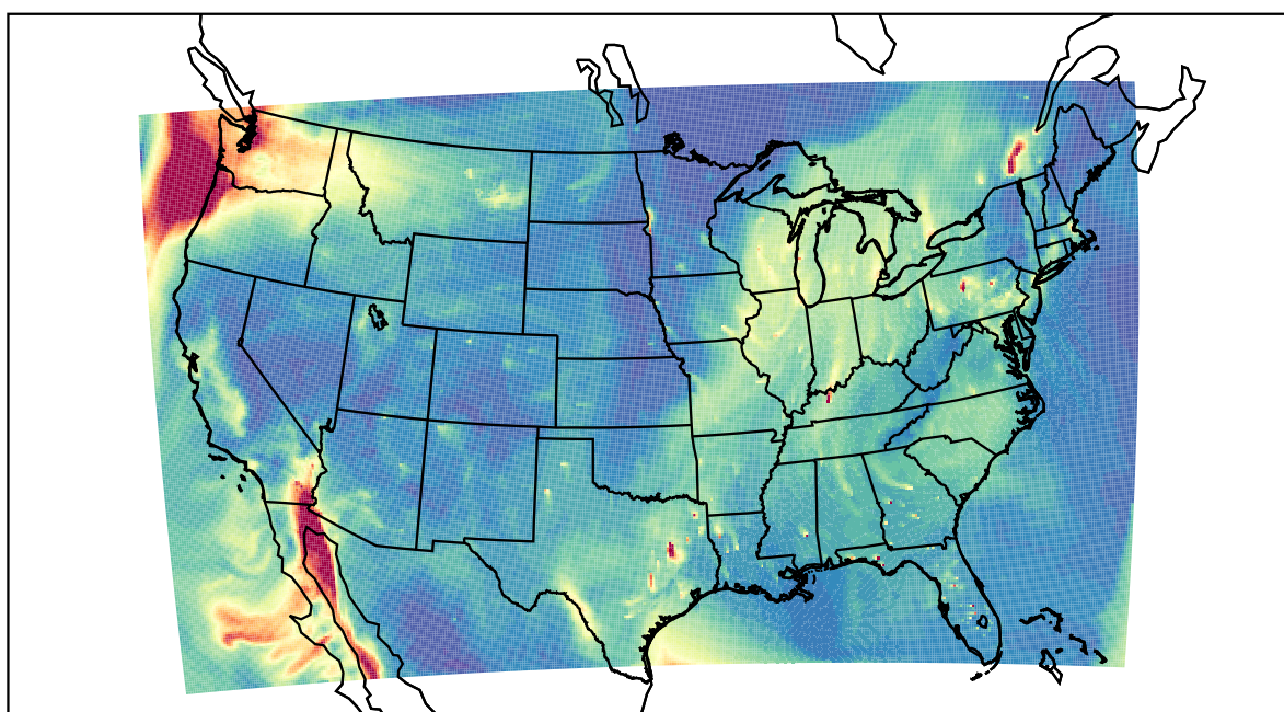
WRF 2020-12-19_18:00:00
