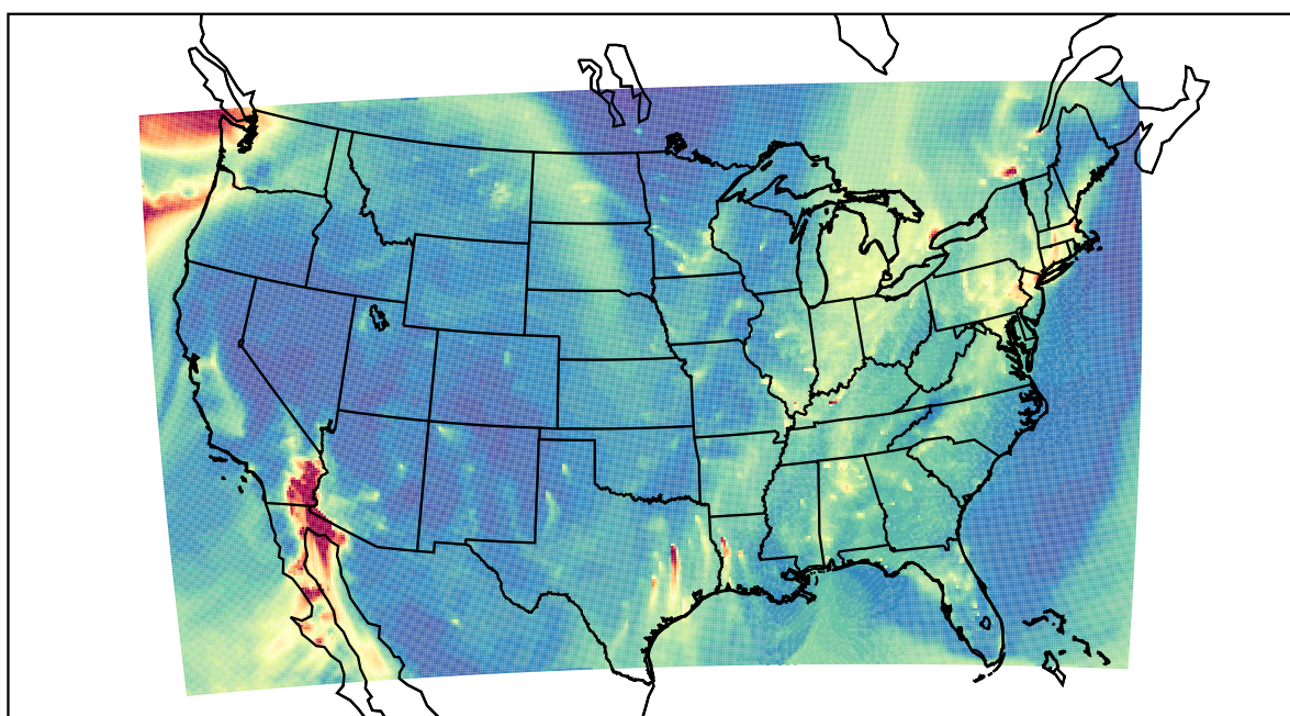
WRF 2020-12-20_13:00:00
