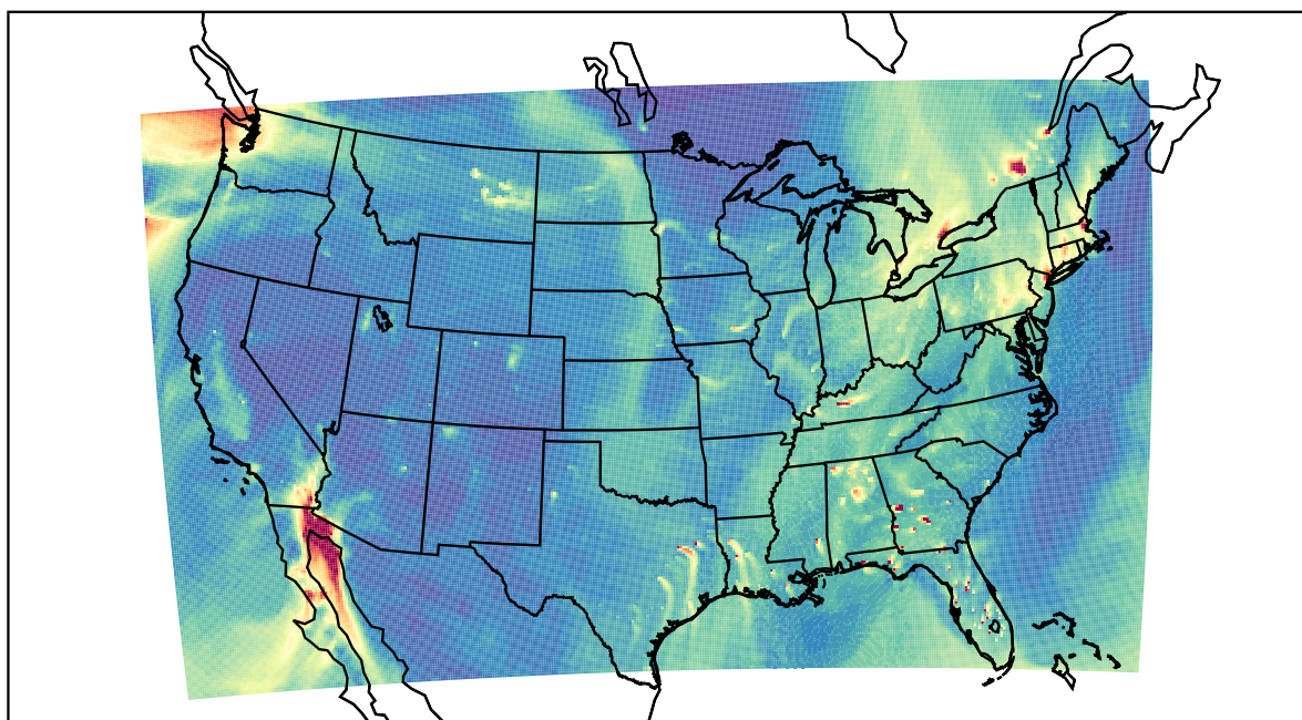
WRF 2020-12-20_20:00:00
