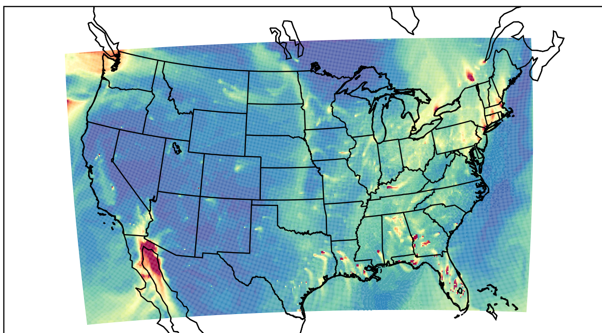
WRF 2020-12-20_23:00:00
