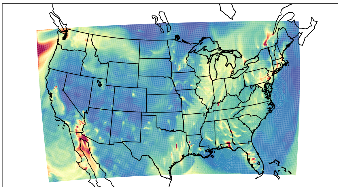
WRF 2020-12-20_03:00:00
