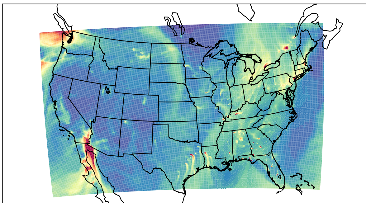
WRF 2020-12-20_18:00:00
