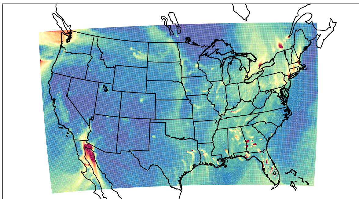
WRF 2020-12-20_22:00:00
