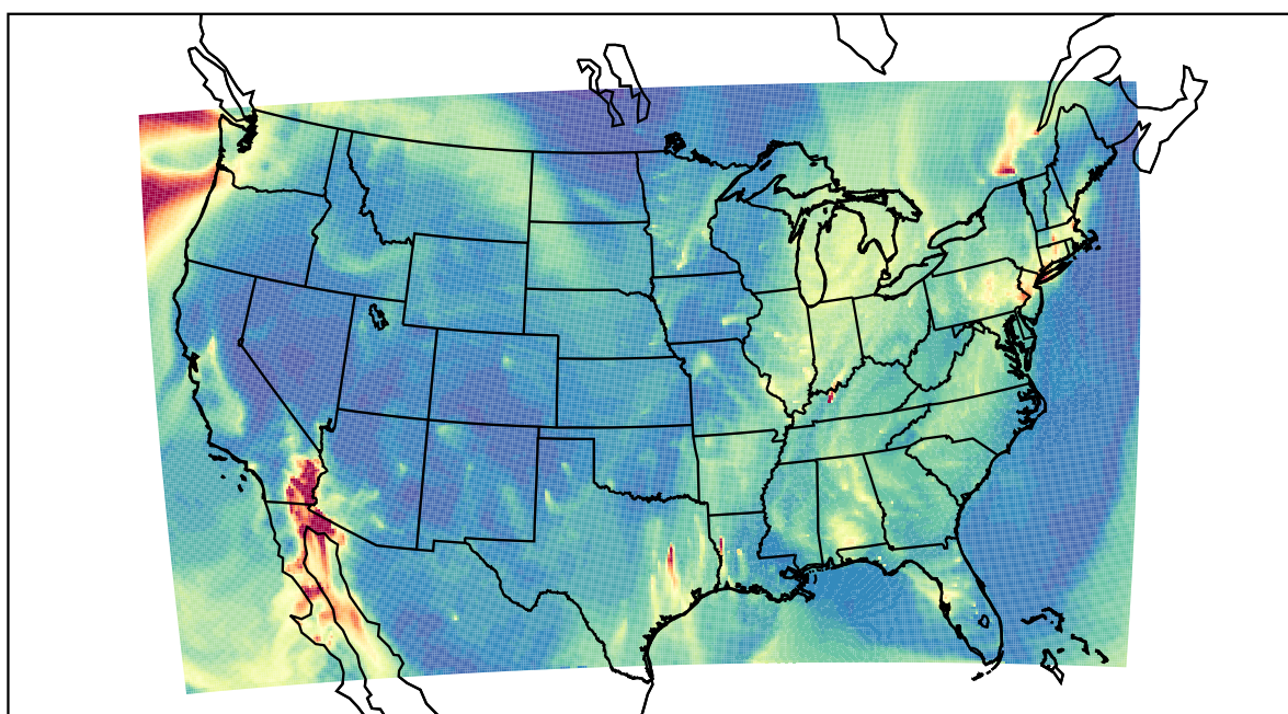
WRF 2020-12-20_08:00:00
