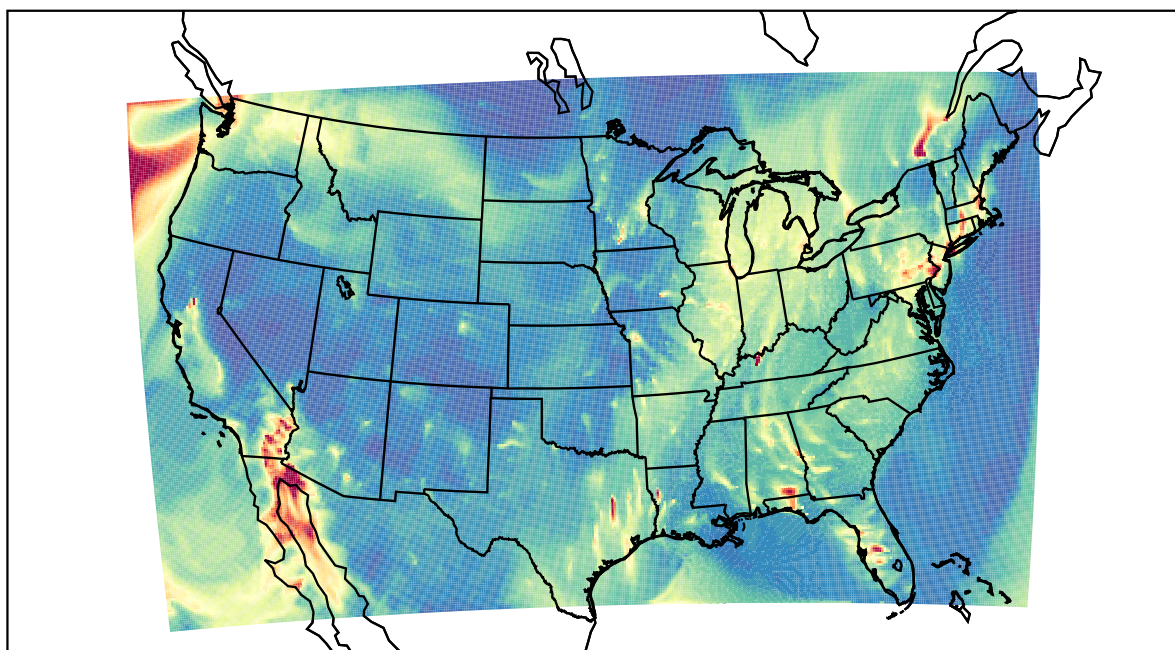
WRF 2020-12-20_04:00:00
