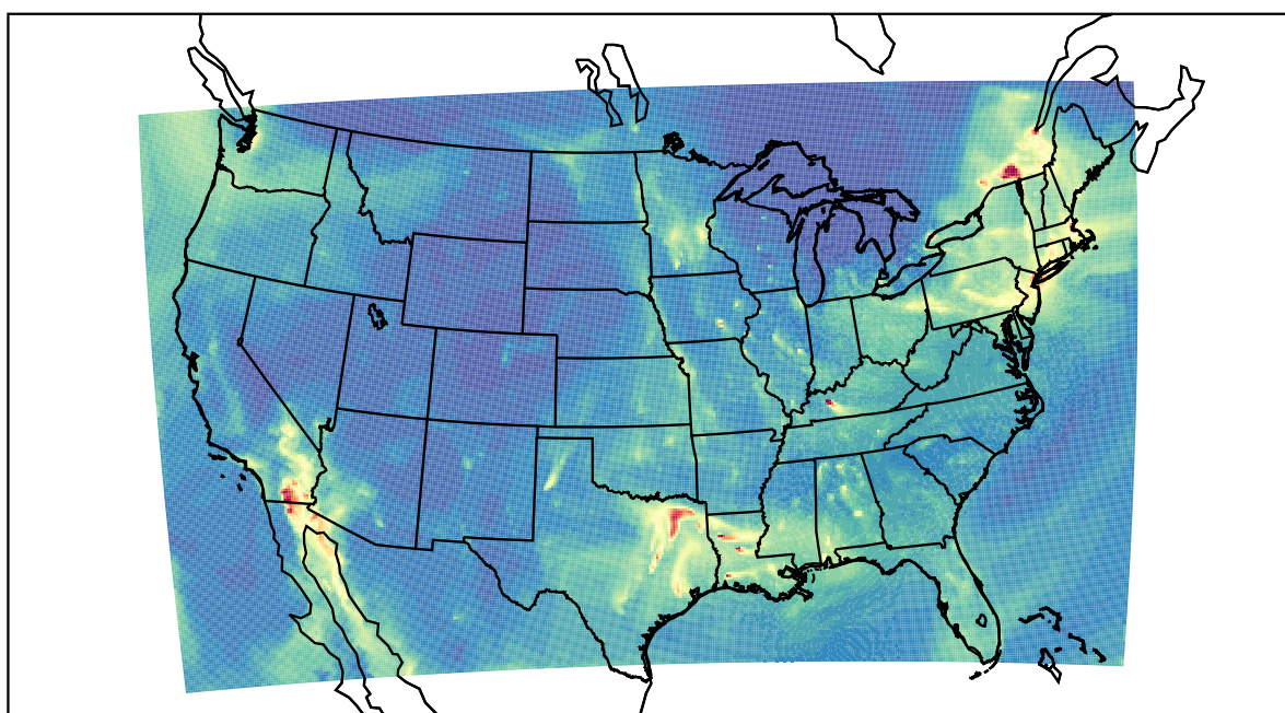
WRF 2020-12-22_14:00:00
