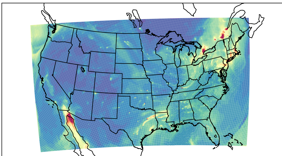
WRF 2020-12-21_22:00:00
