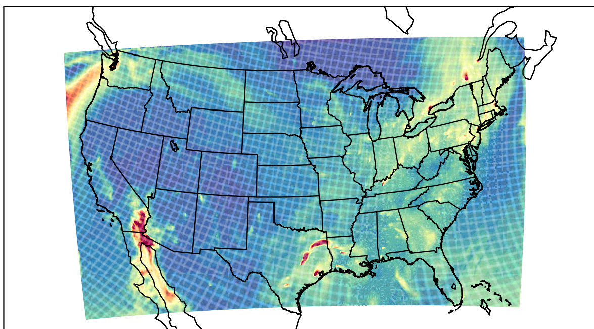
WRF 2020-12-21_13:00:00
