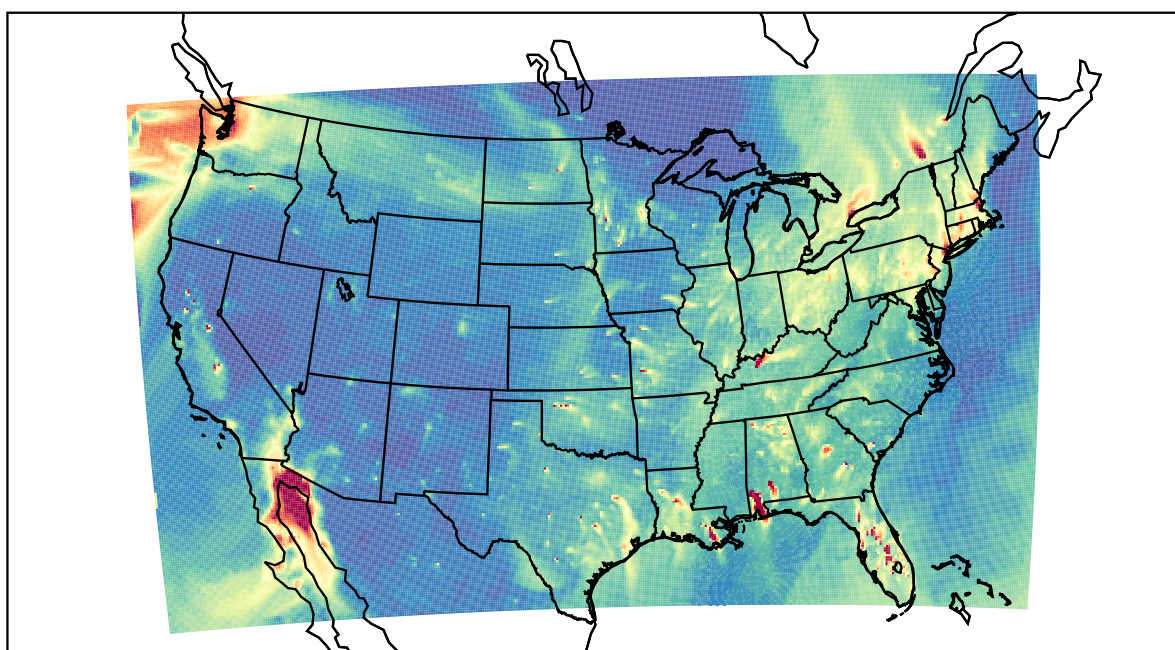
WRF 2020-12-21_00:00:00
