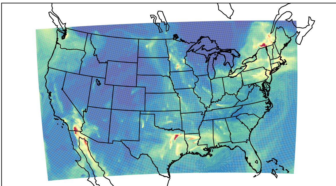
WRF 2020-12-22_10:00:00
