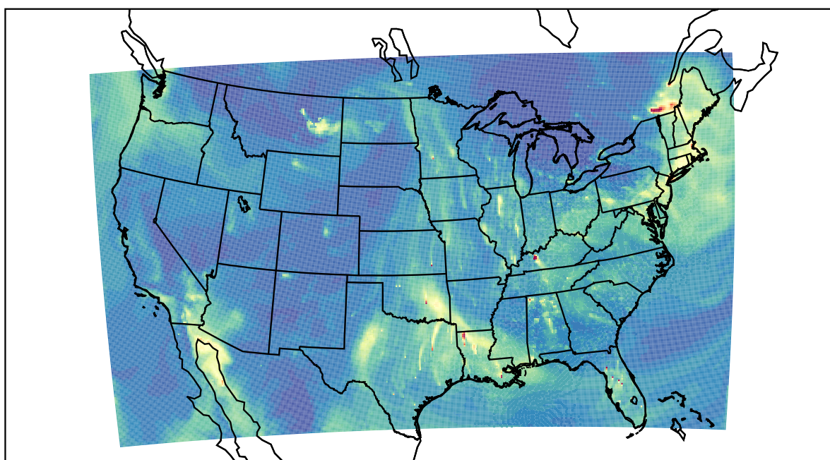
WRF 2020-12-22_22:00:00
