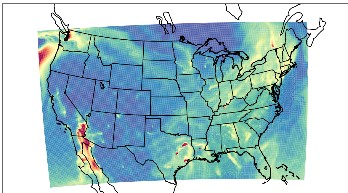
WRF 2020-12-21_09:00:00
