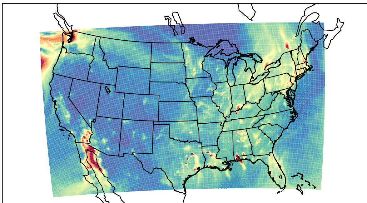
WRF 2020-12-21_04:00:00
