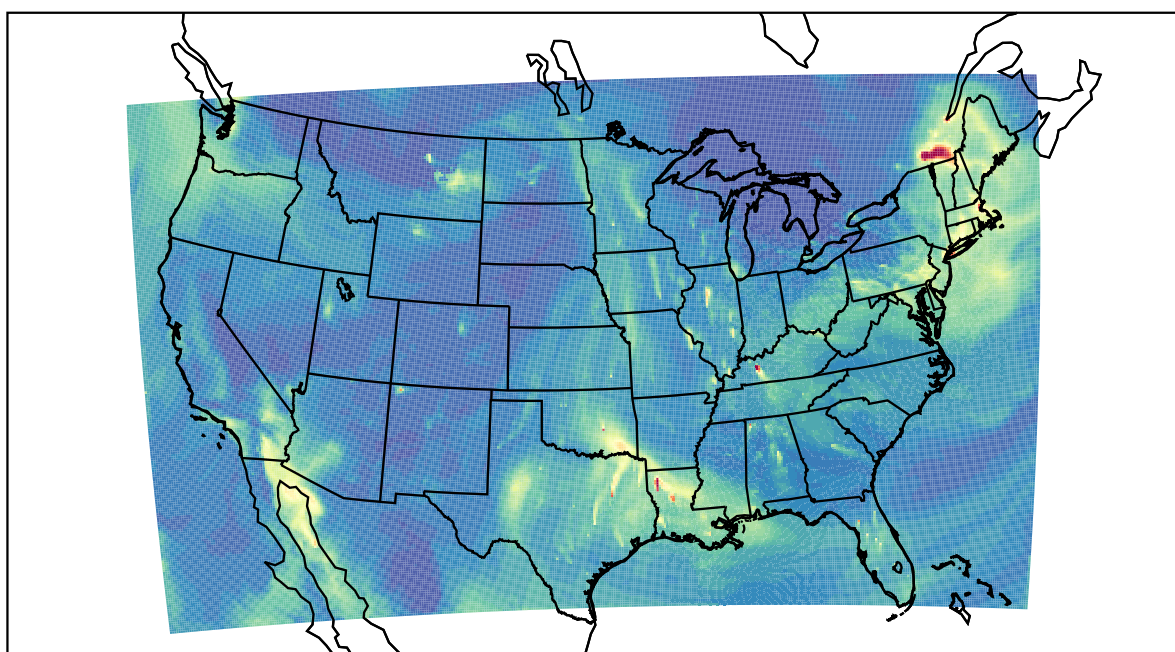
WRF 2020-12-22_20:00:00
