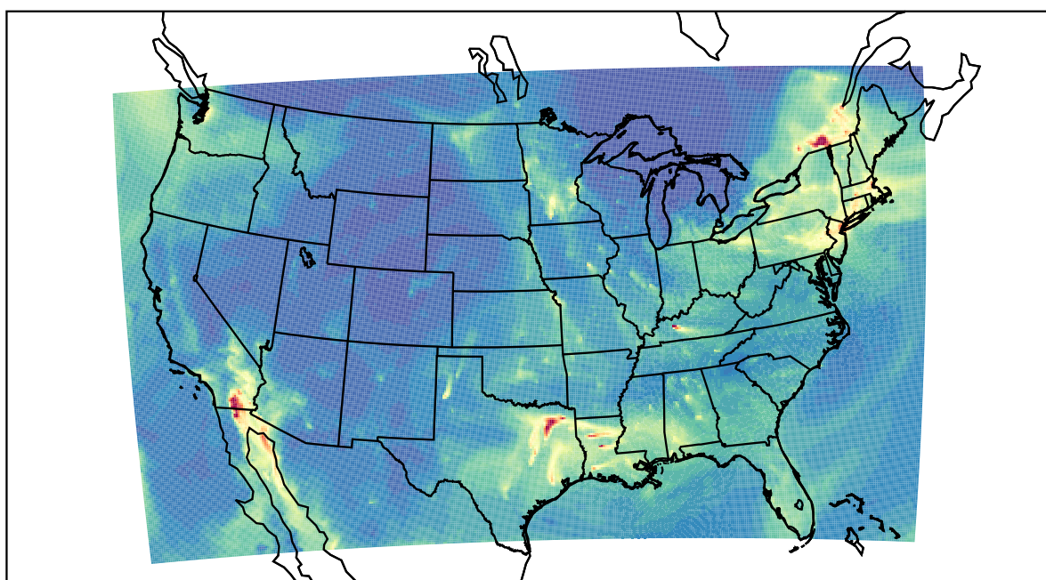
WRF 2020-12-22_12:00:00
