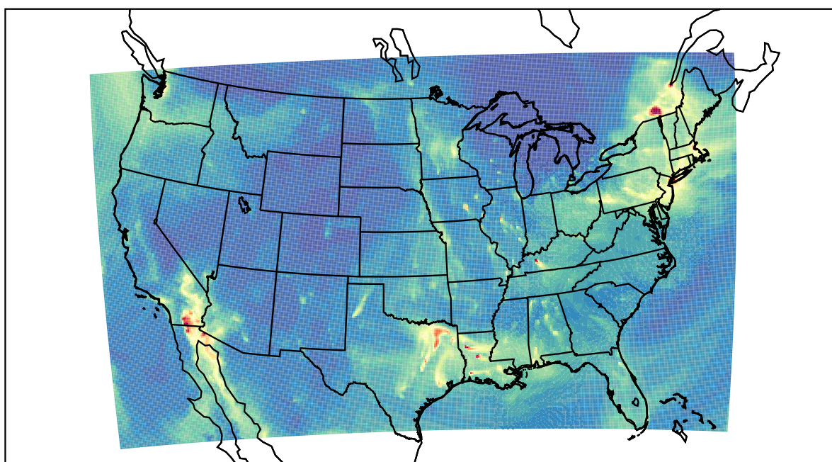
WRF 2020-12-22_15:00:00
