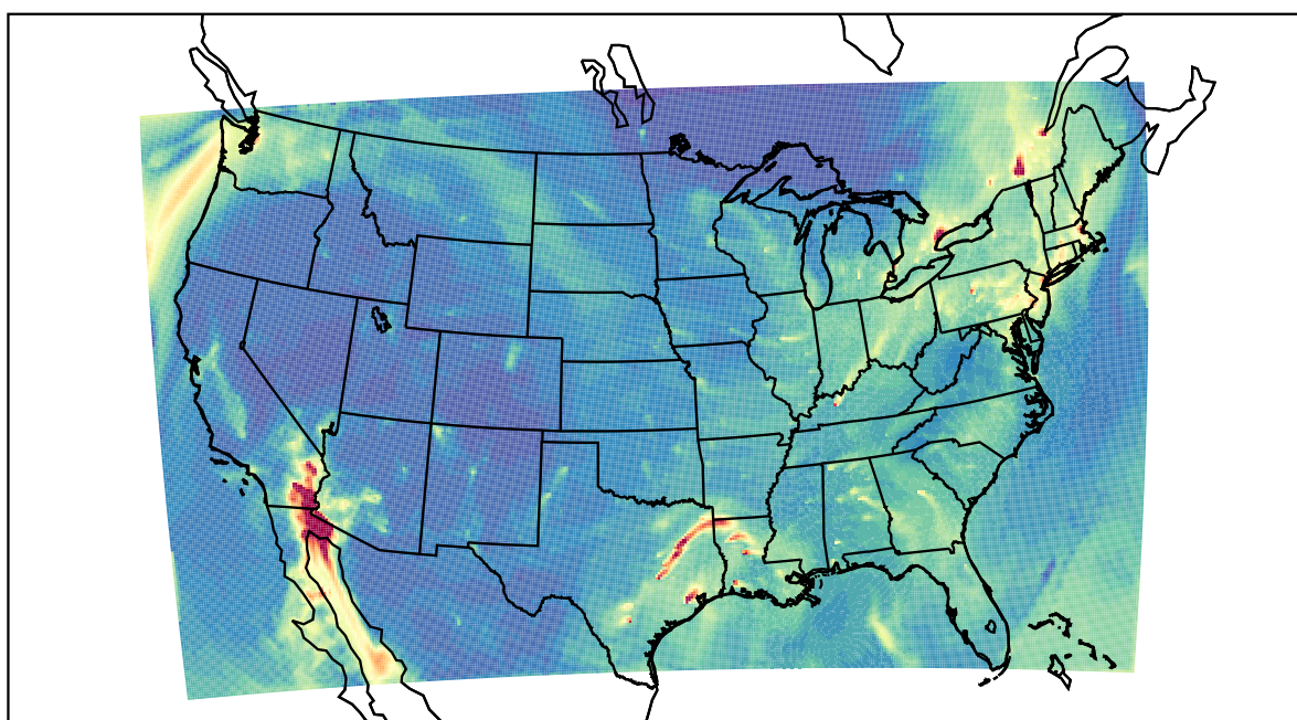
WRF 2020-12-21_16:00:00
