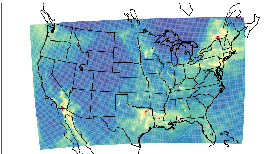
WRF 2020-12-22_13:00:00
