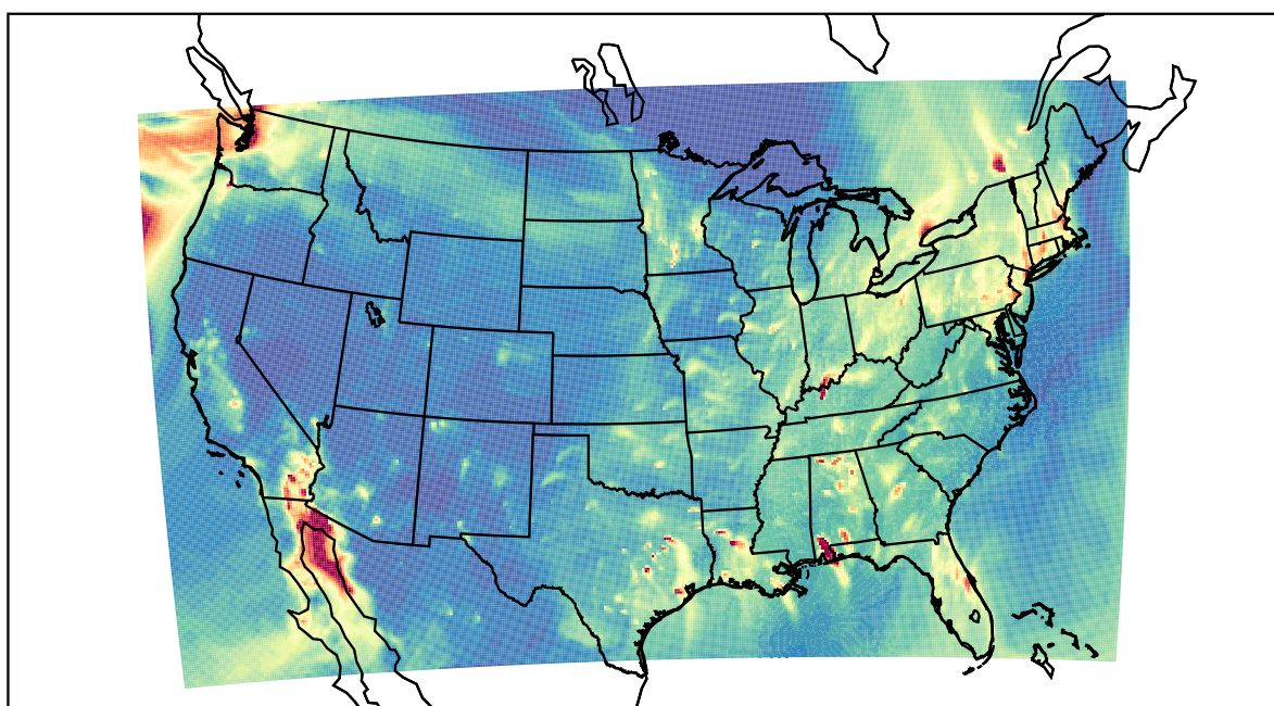
WRF 2020-12-21_03:00:00
