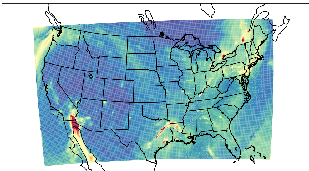
WRF 2020-12-21_17:00:00
