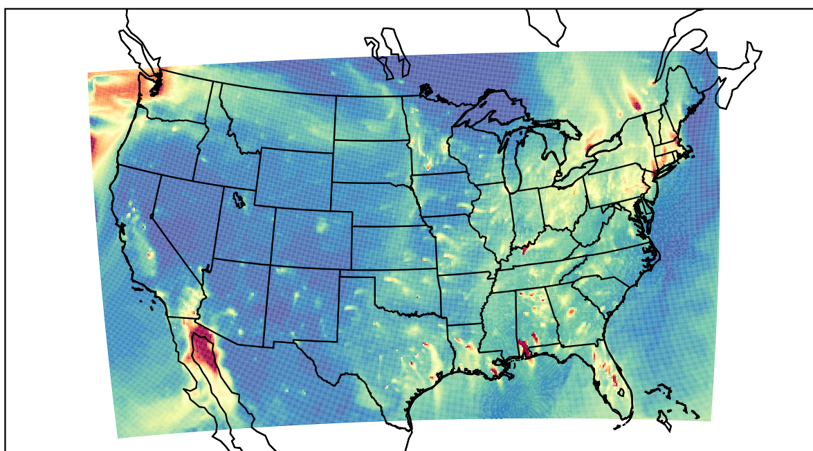
WRF 2020-12-21_01:00:00
