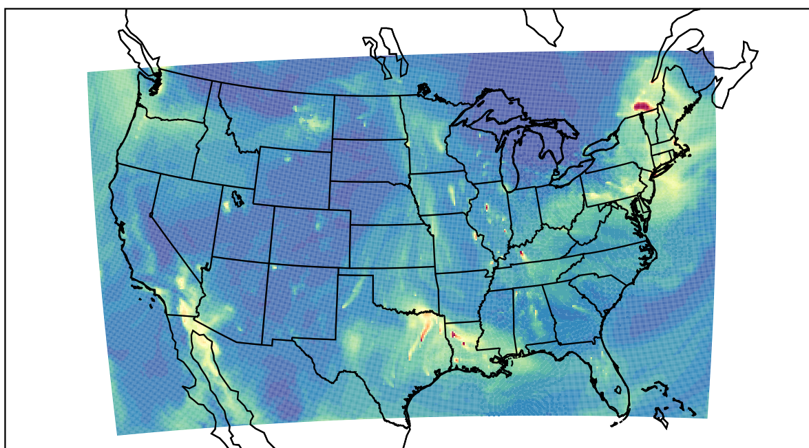
WRF 2020-12-22_18:00:00
