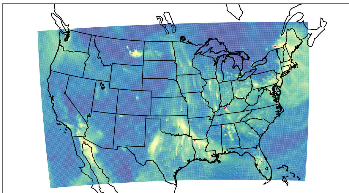
WRF 2020-12-22_23:00:00
