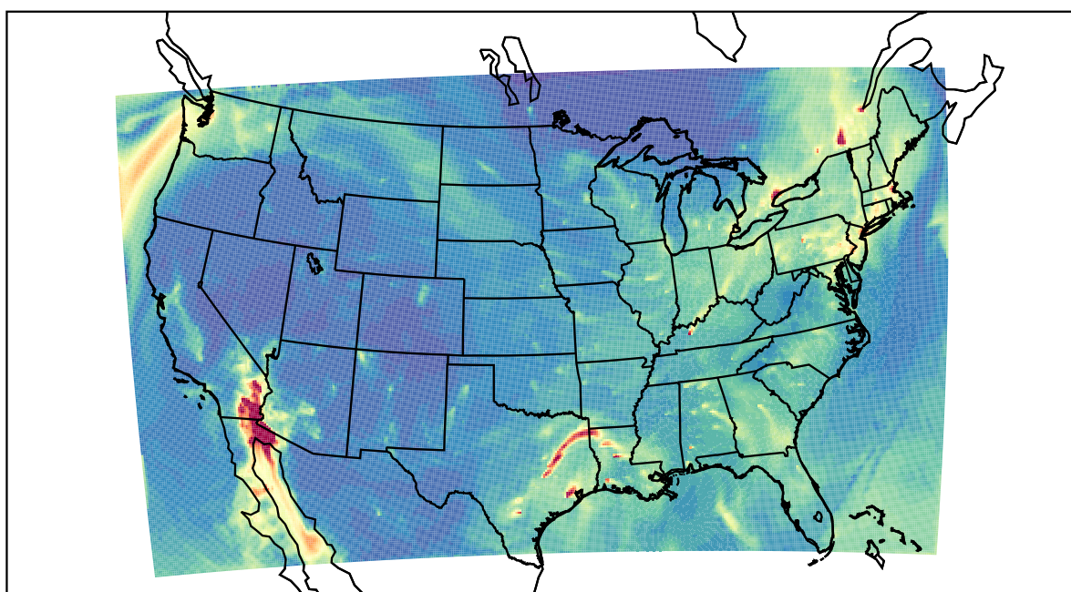
WRF 2020-12-21_15:00:00
