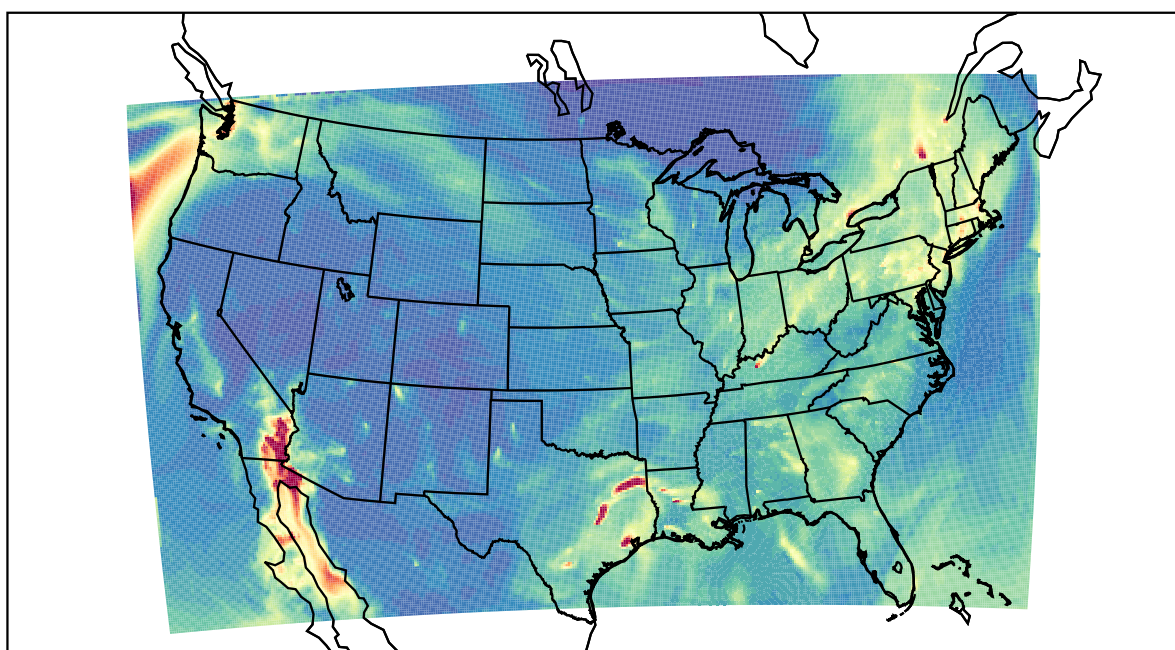
WRF 2020-12-21_12:00:00
