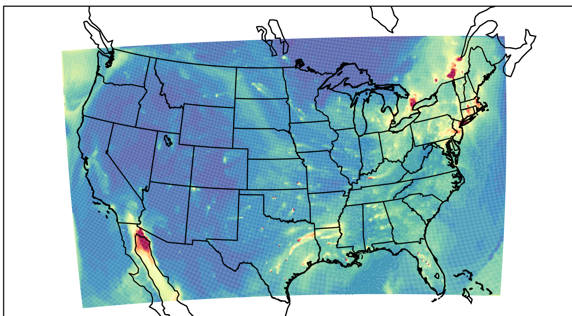
WRF 2020-12-21_23:00:00
