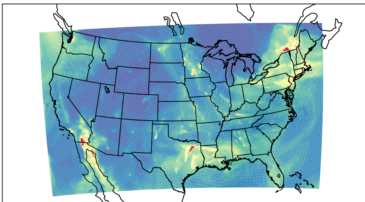
WRF 2020-12-22_11:00:00
