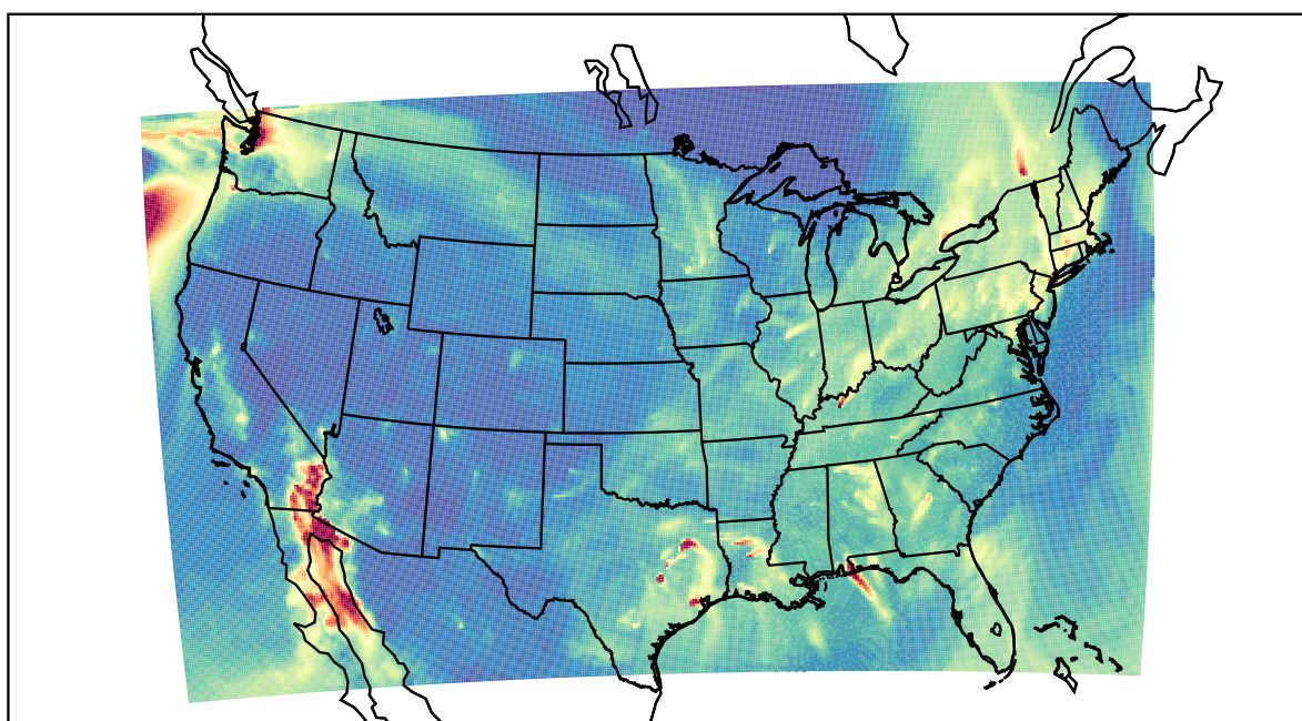
WRF 2020-12-21_07:00:00
