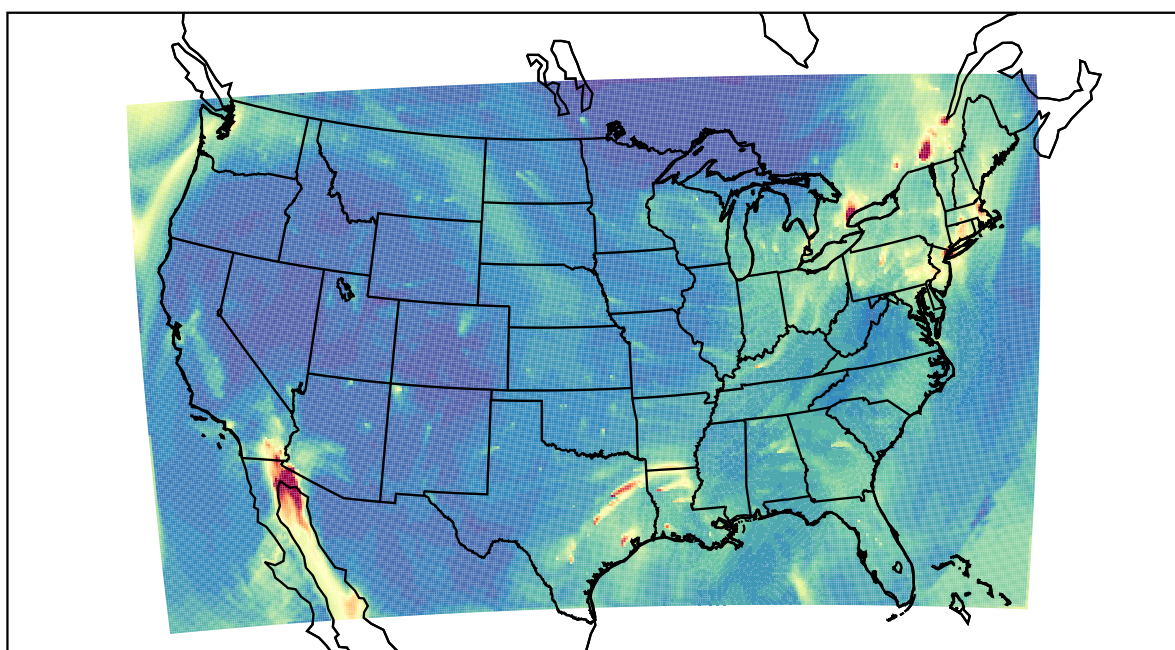
WRF 2020-12-21_19:00:00
