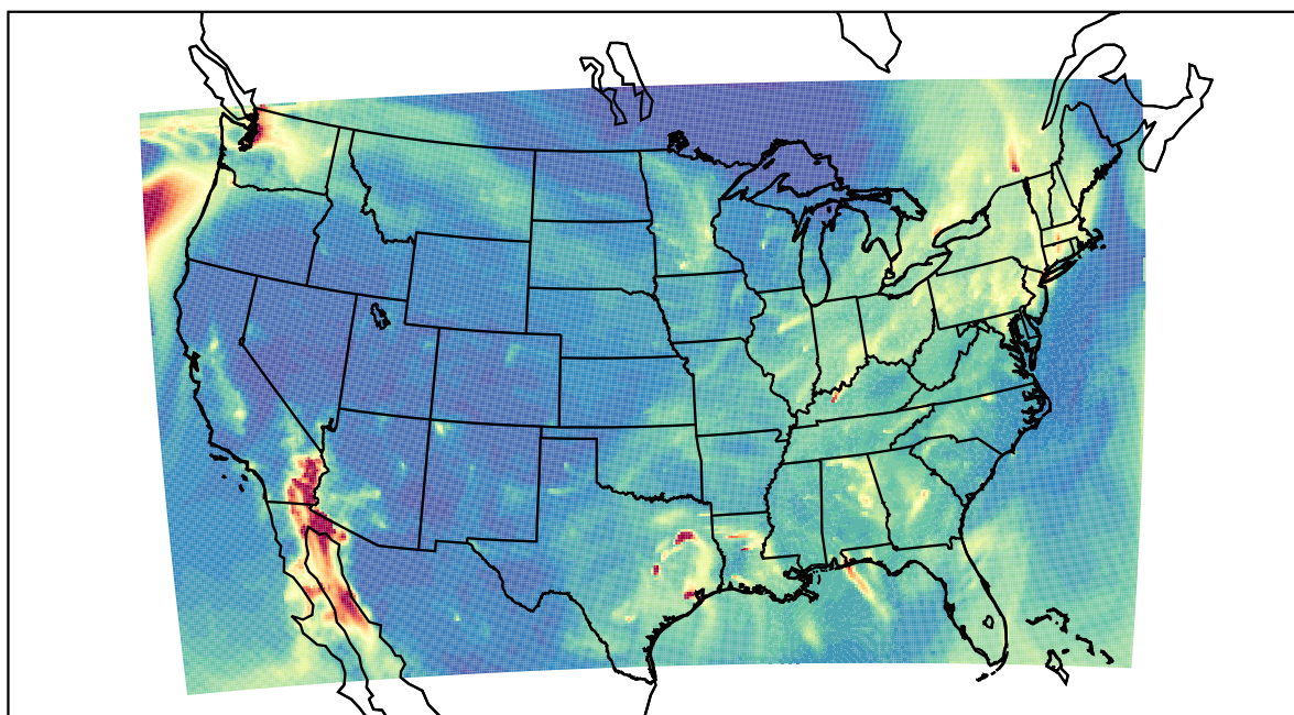
WRF 2020-12-21_08:00:00
