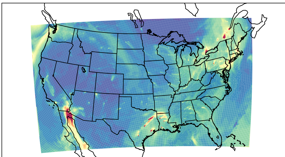
WRF 2020-12-21_18:00:00
