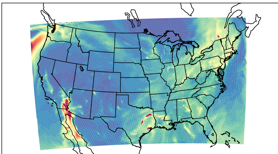
WRF 2020-12-21_11:00:00
