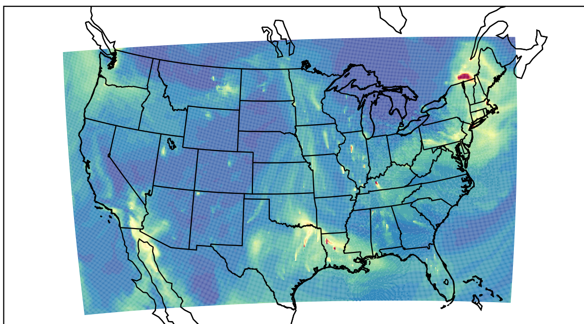
WRF 2020-12-22_19:00:00
