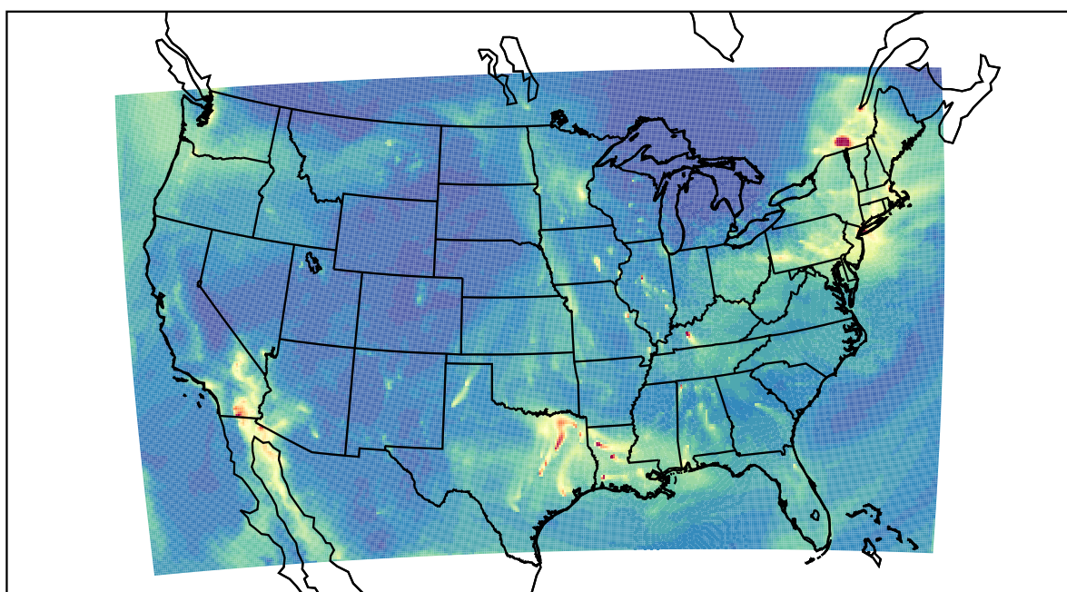
WRF 2020-12-22_16:00:00
