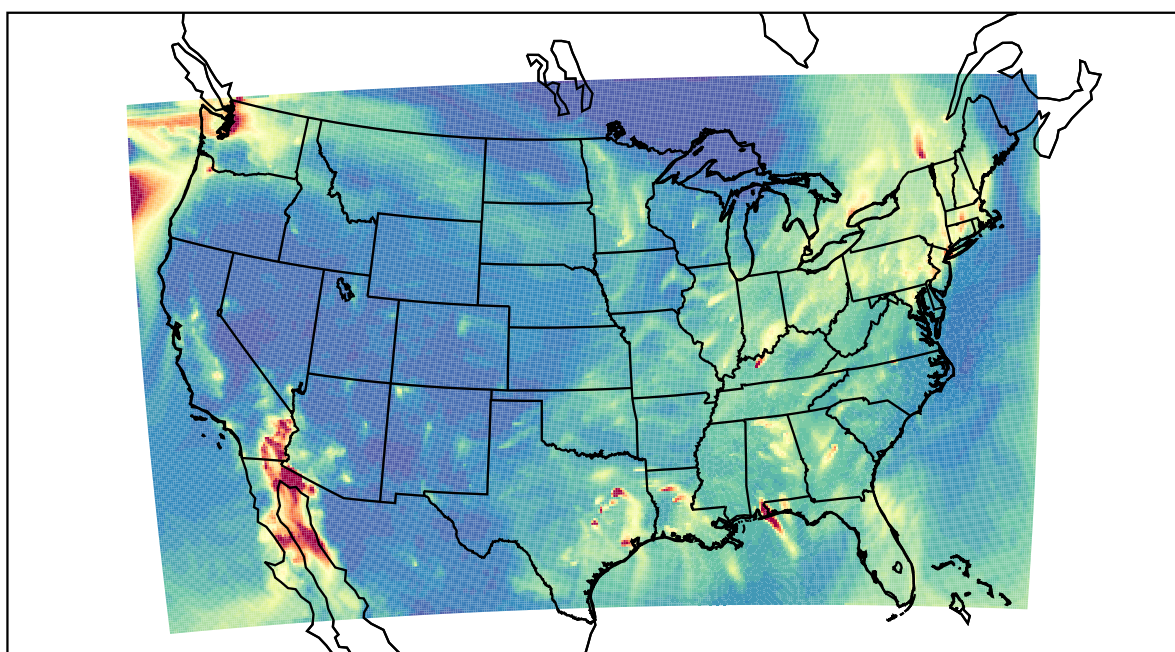
WRF 2020-12-21_06:00:00
