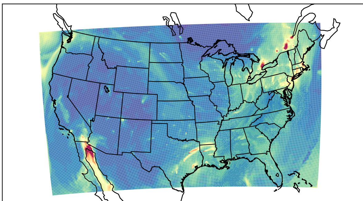
WRF 2020-12-21_20:00:00
