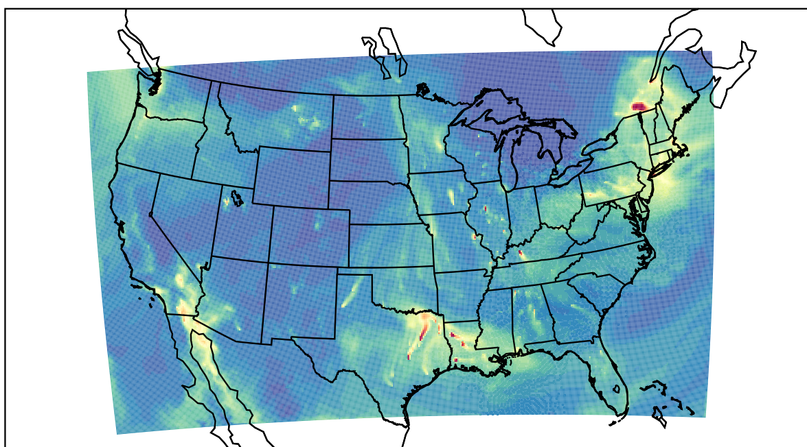
WRF 2020-12-22_17:00:00
