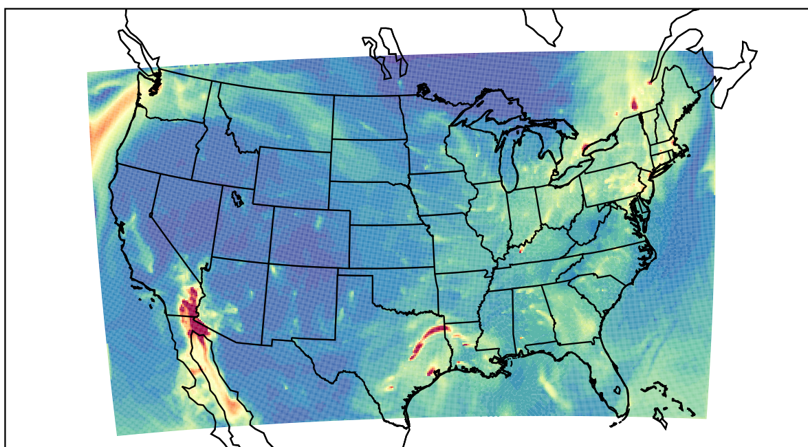
WRF 2020-12-21_14:00:00
