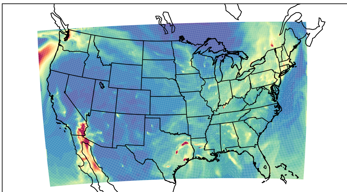
WRF 2020-12-21_10:00:00
