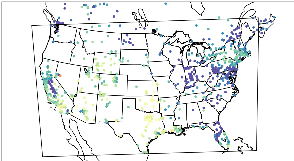
AirNOW (2020-12-22_23:00:00)
