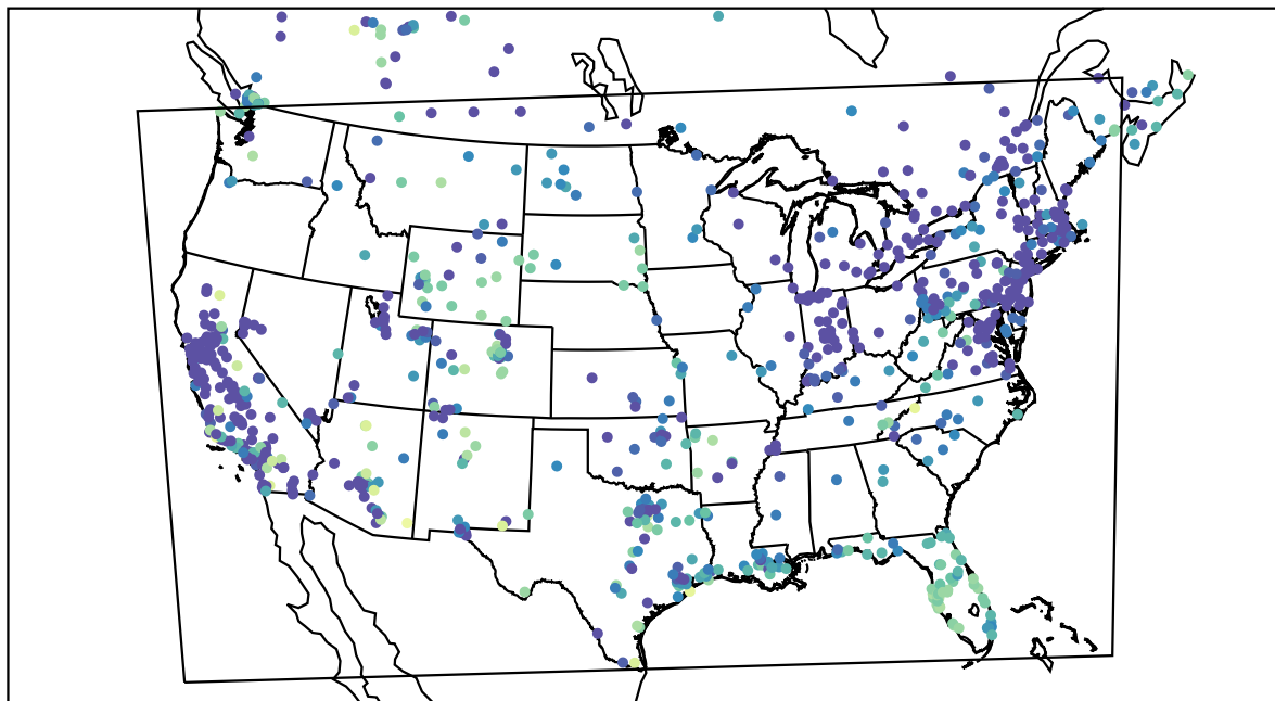
AirNOW (2020-12-21_16:00:00)
