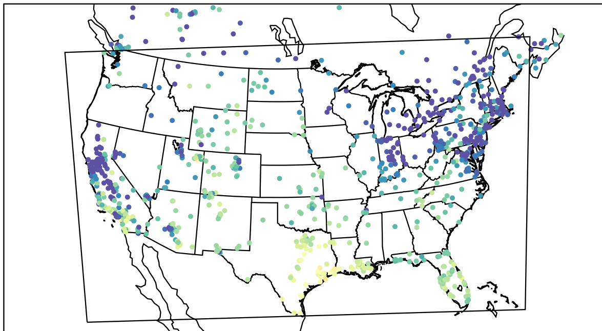
AirNOW (2020-12-21_19:00:00)
