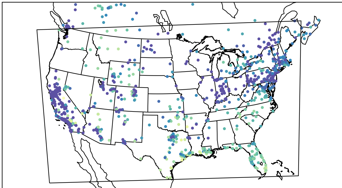
AirNOW (2020-12-22_16:00:00)
