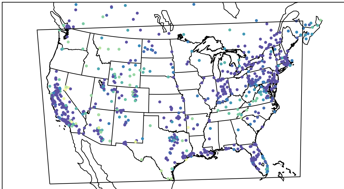
AirNOW (2020-12-22_10:00:00)
