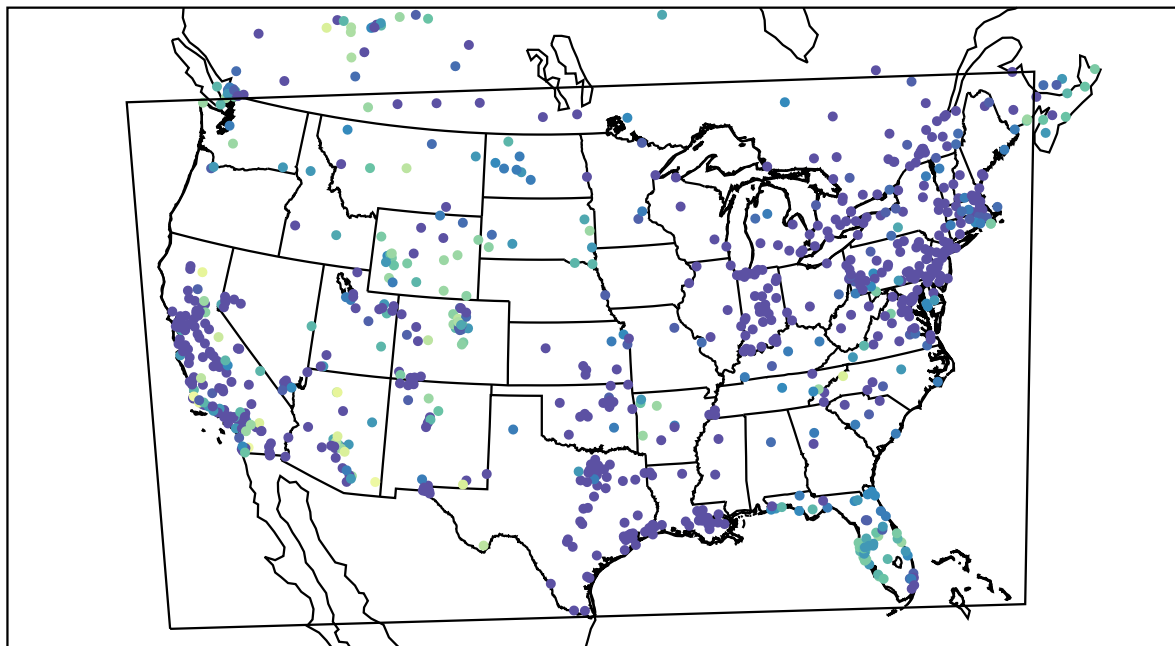
AirNOW (2020-12-21_14:00:00)
