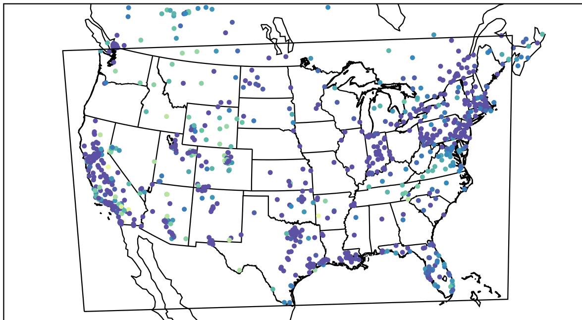
AirNOW (2020-12-22_14:00:00)
