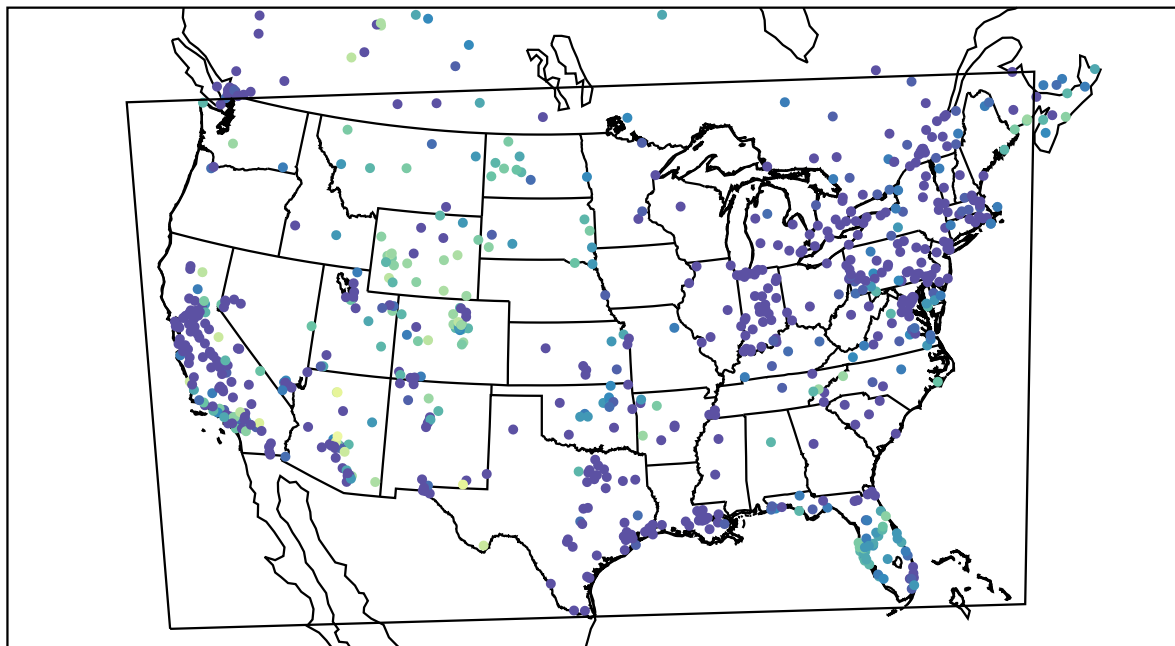
AirNOW (2020-12-21_10:00:00)
