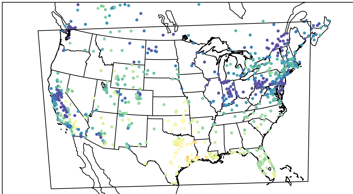
AirNOW (2020-12-22_19:00:00)
