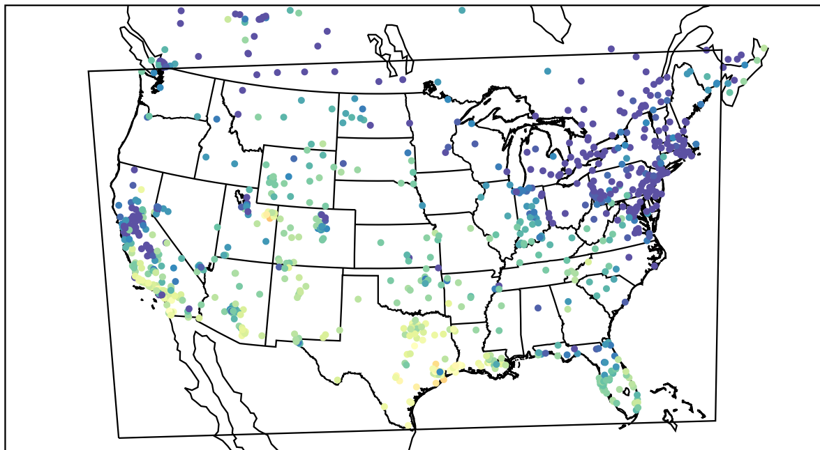
AirNOW (2020-12-21_22:00:00)
