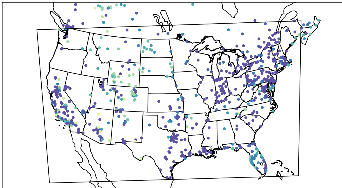
AirNOW (2020-12-21_11:00:00)
