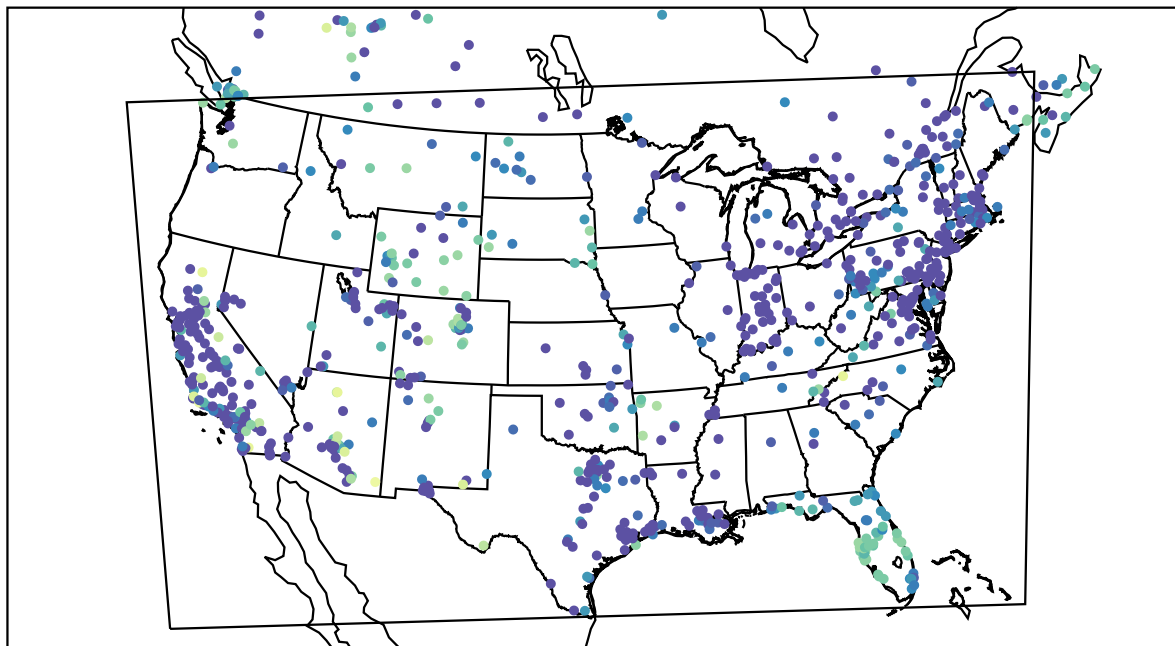
AirNOW (2020-12-21_15:00:00)
