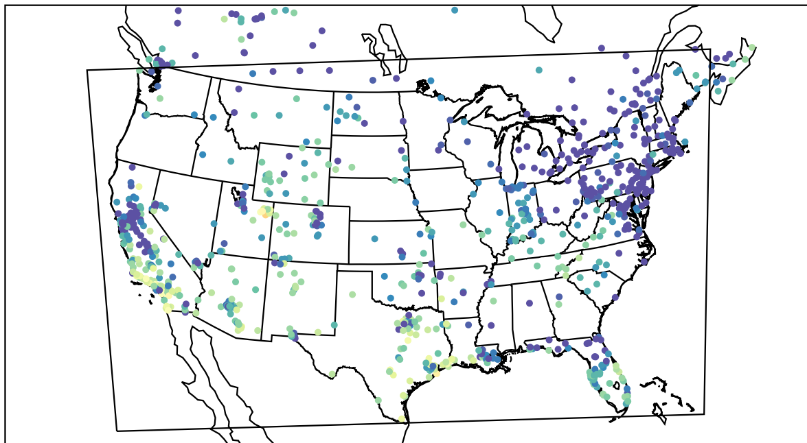
AirNOW (2020-12-21_23:00:00)
