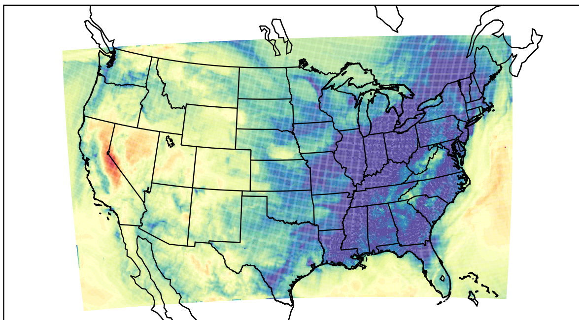
WRF (2020-12-21_11:00:00)
