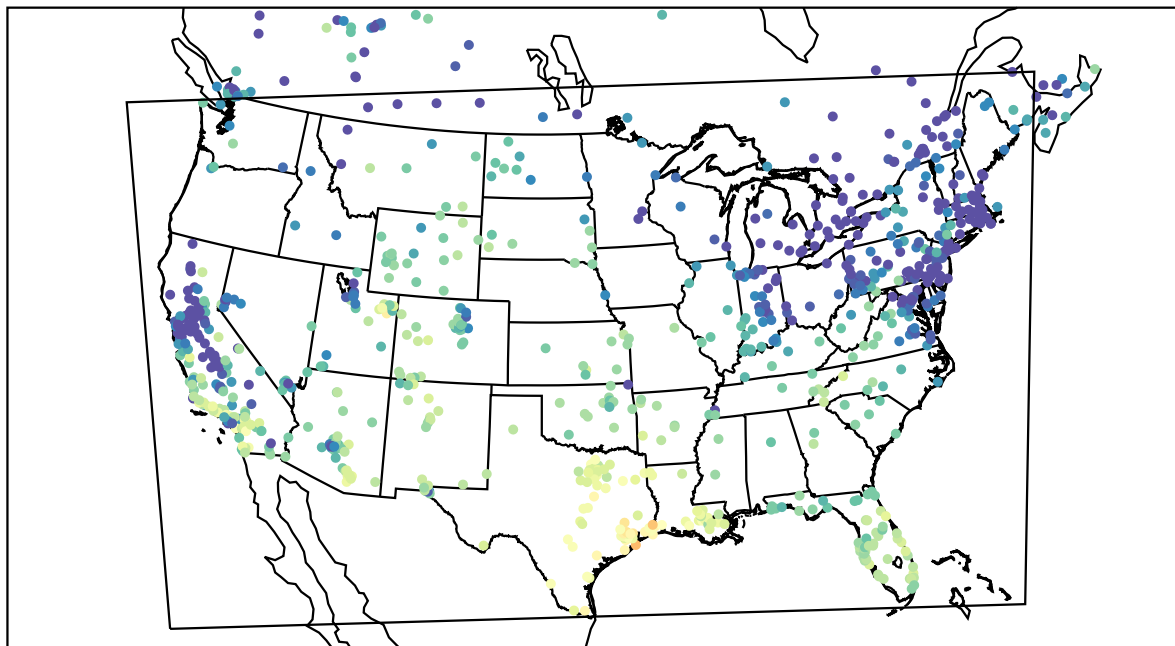
AirNOW (2020-12-21_20:00:00)
