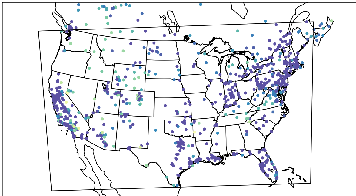
AirNOW (2020-12-22_13:00:00)
