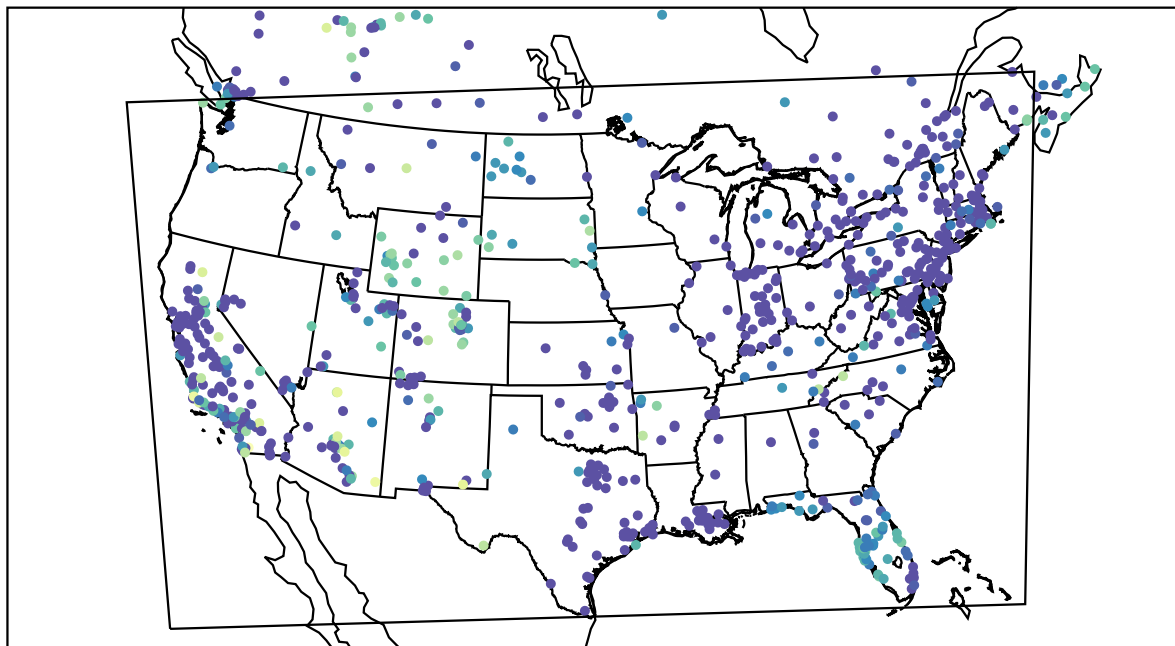
AirNOW (2020-12-21_13:00:00)
