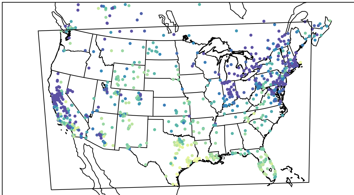
AirNOW (2020-12-21_18:00:00)
