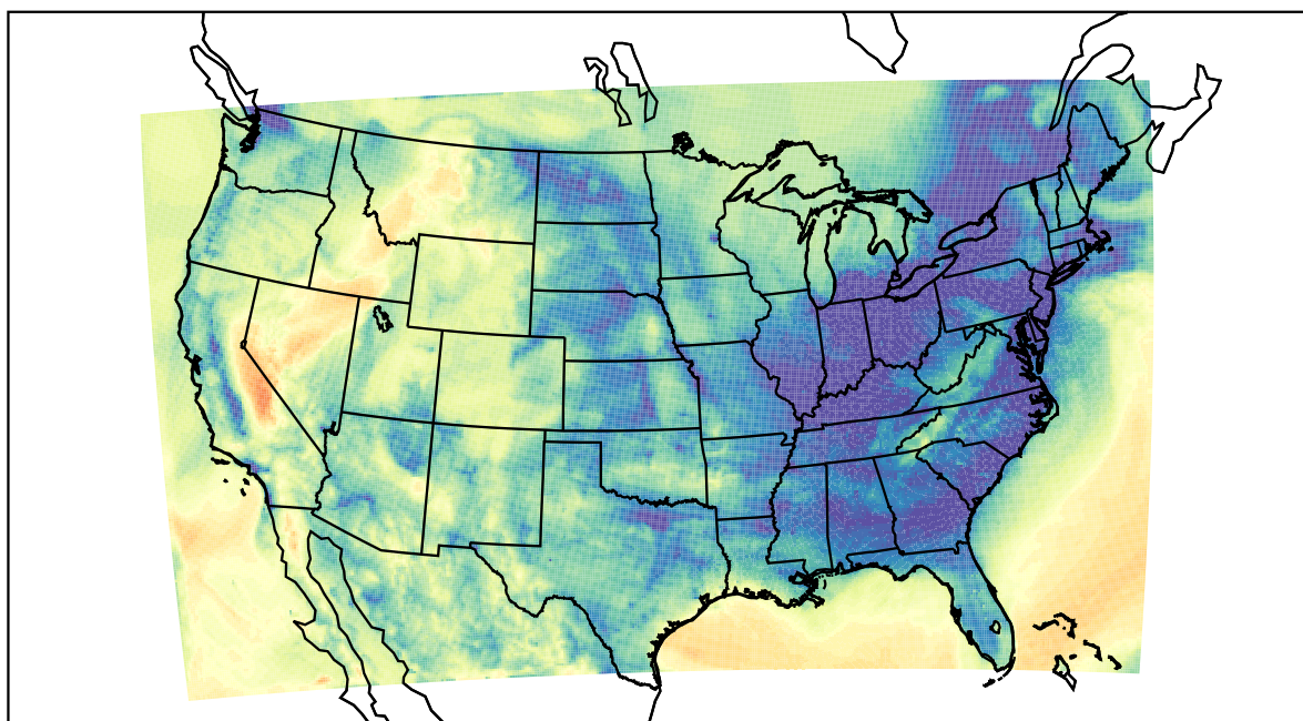
WRF (2020-12-22_10:00:00)
