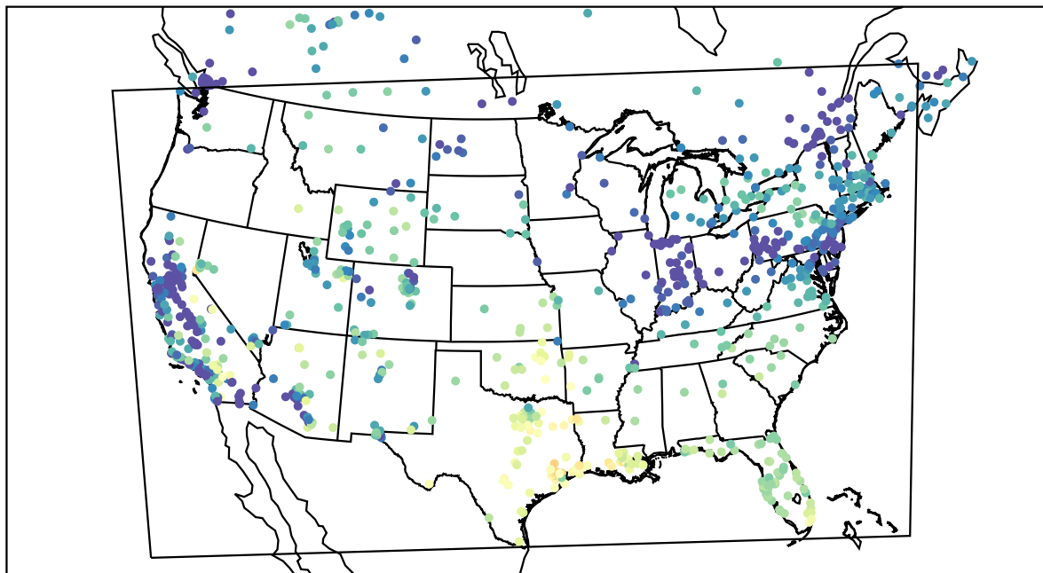
AirNOW (2020-12-22_18:00:00)
