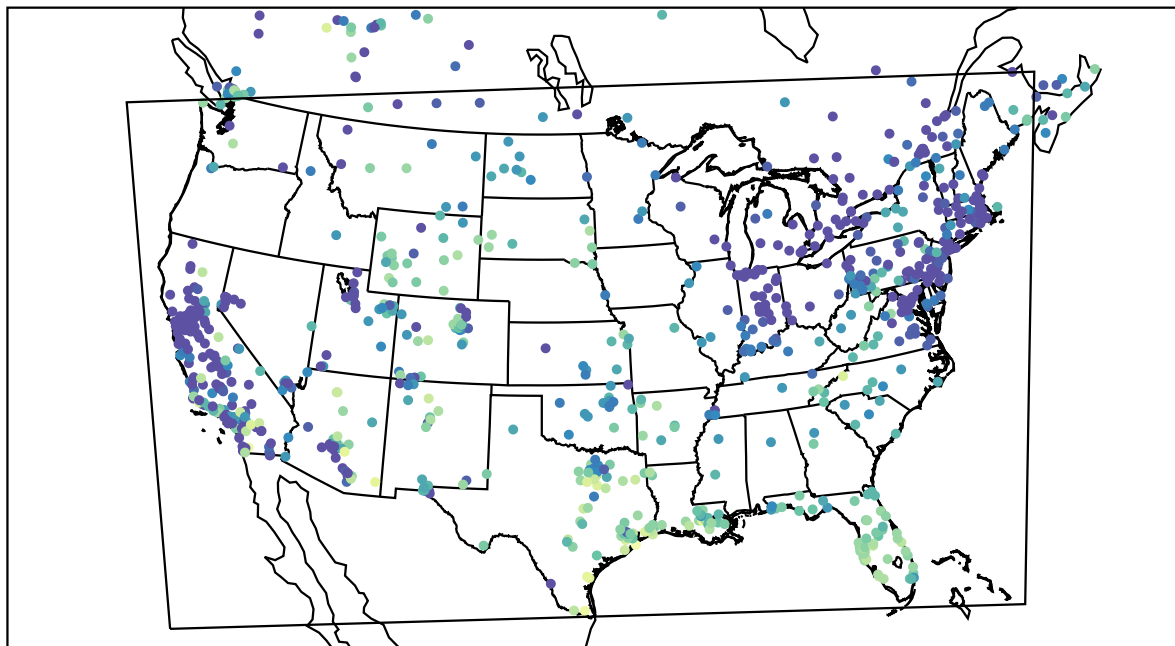
AirNOW (2020-12-21_17:00:00)
