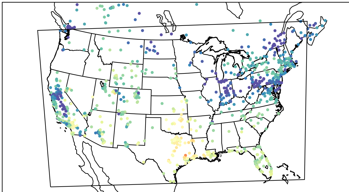
AirNOW (2020-12-22_20:00:00)
