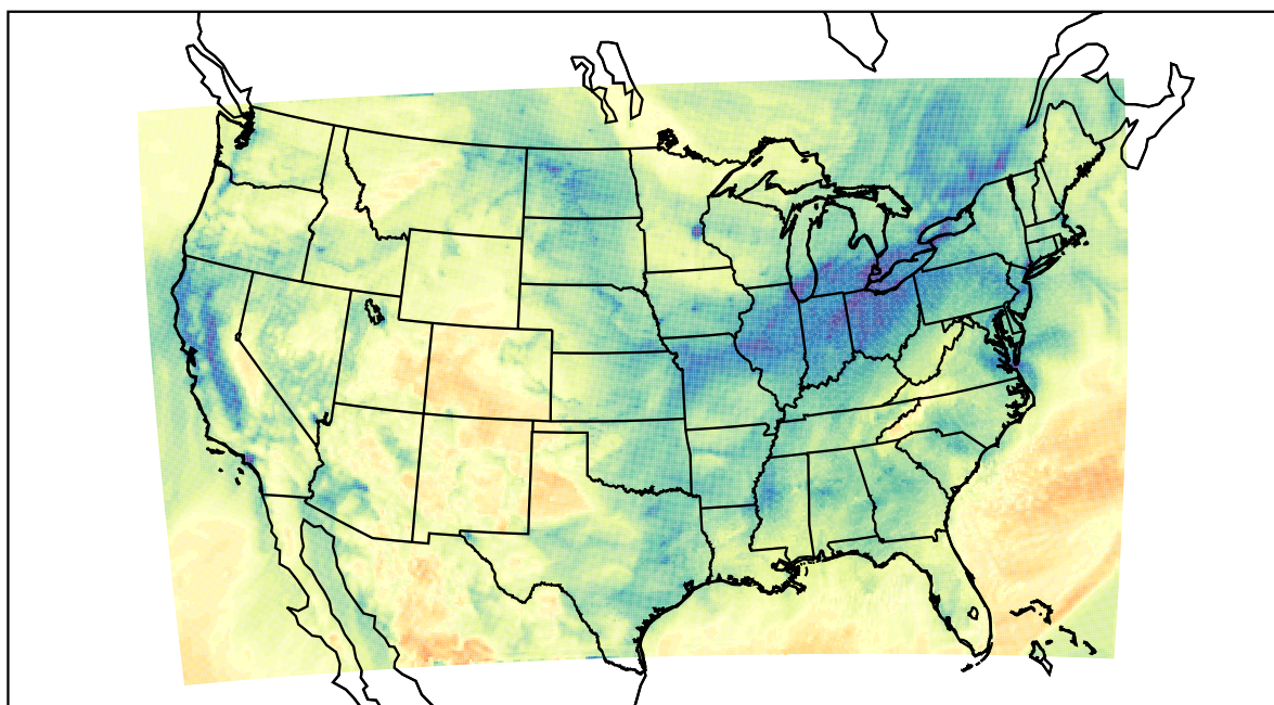
WRF (2021-01-13_18:00:00)
