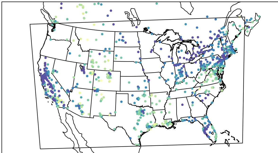
AirNOW (2021-01-13_18:00:00)
