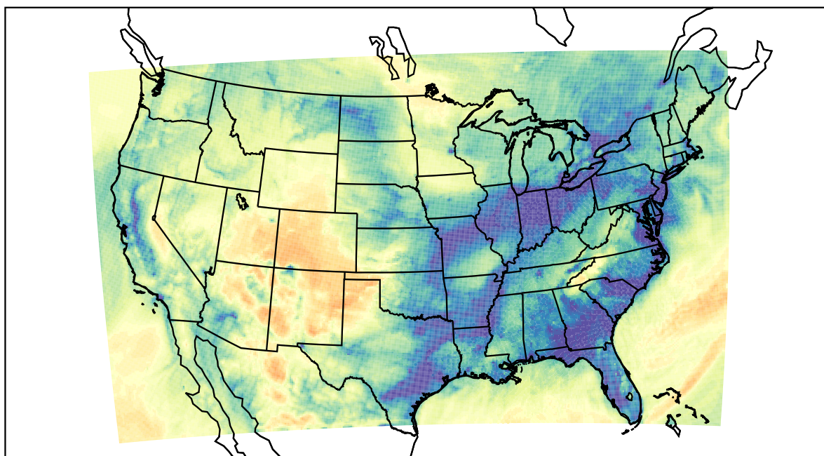
WRF (2021-01-13_13:00:00)
