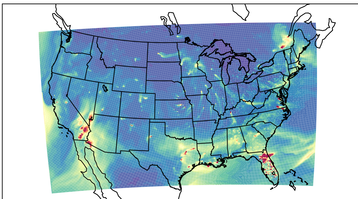
WRF 2021-01-22_23:00:00
