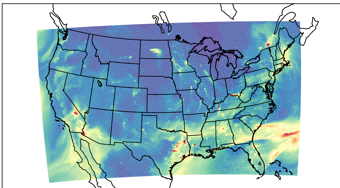
WRF 2021-01-22_14:00:00
