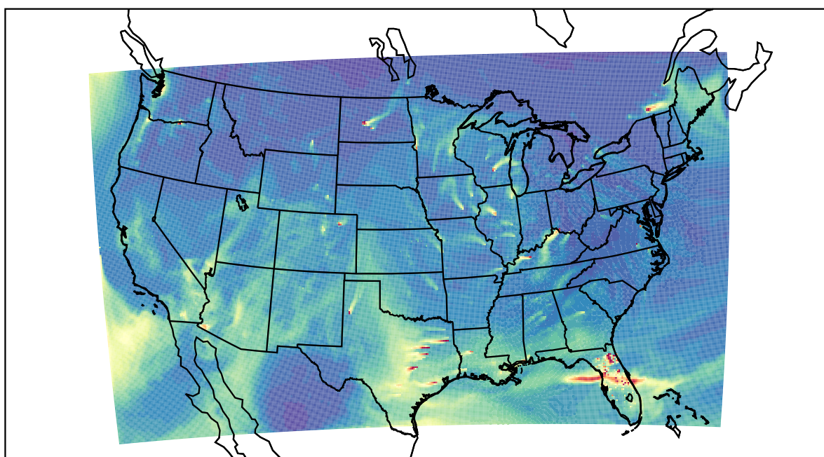
WRF 2021-01-23_18:00:00
