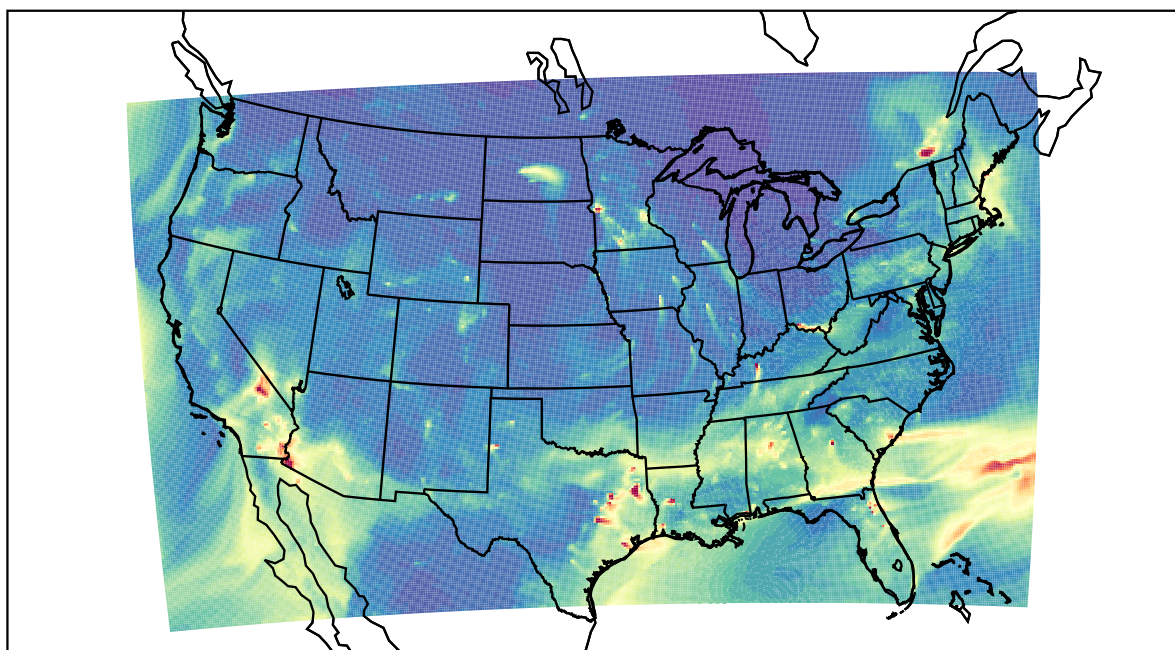
WRF 2021-01-22_15:00:00
