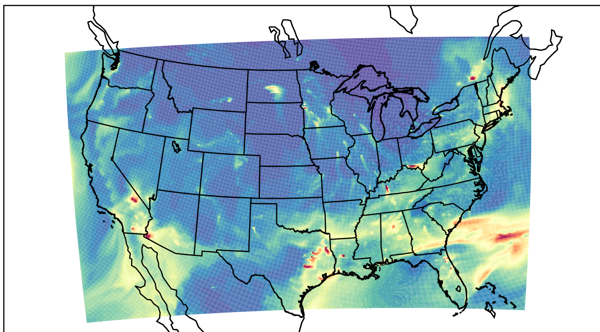
WRF 2021-01-22_13:00:00
