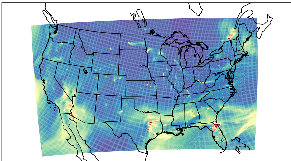
WRF 2021-01-22_20:00:00
