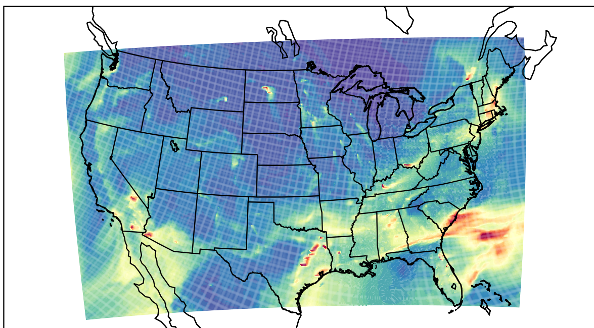
WRF 2021-01-22_10:00:00
