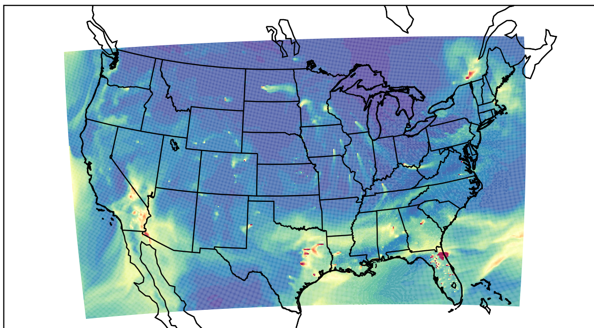
WRF 2021-01-22_19:00:00
