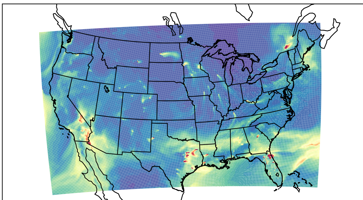
WRF 2021-01-22_18:00:00
