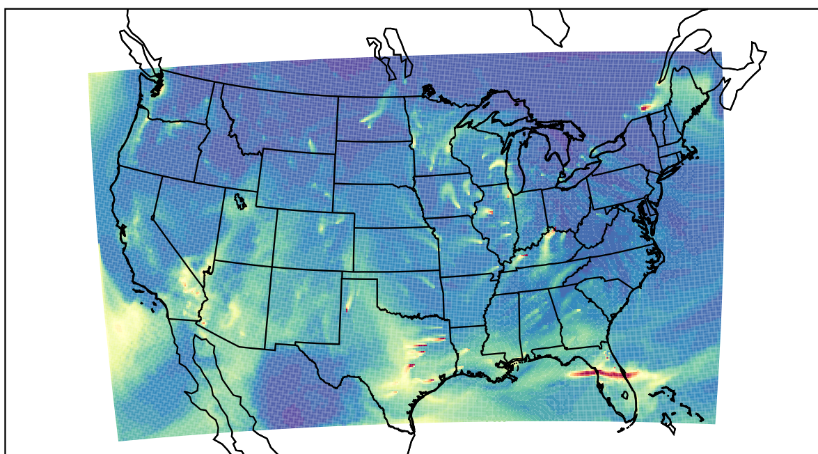
WRF 2021-01-23_16:00:00
