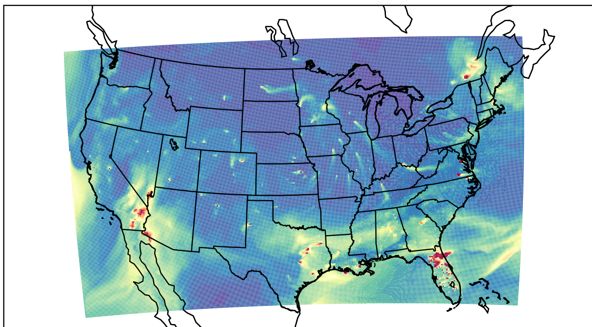
WRF 2021-01-22_22:00:00
