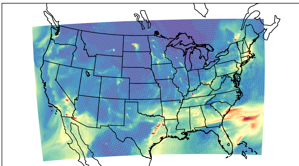
WRF 2021-01-22_11:00:00
