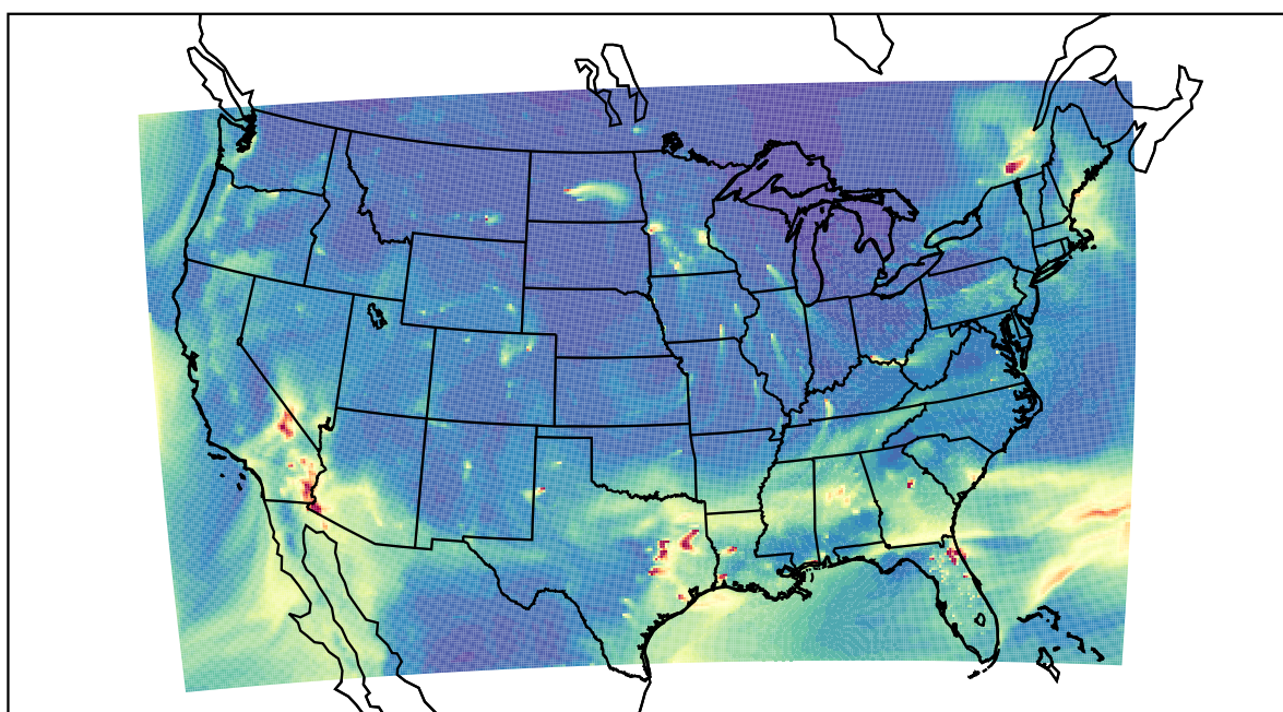
WRF 2021-01-22_17:00:00
