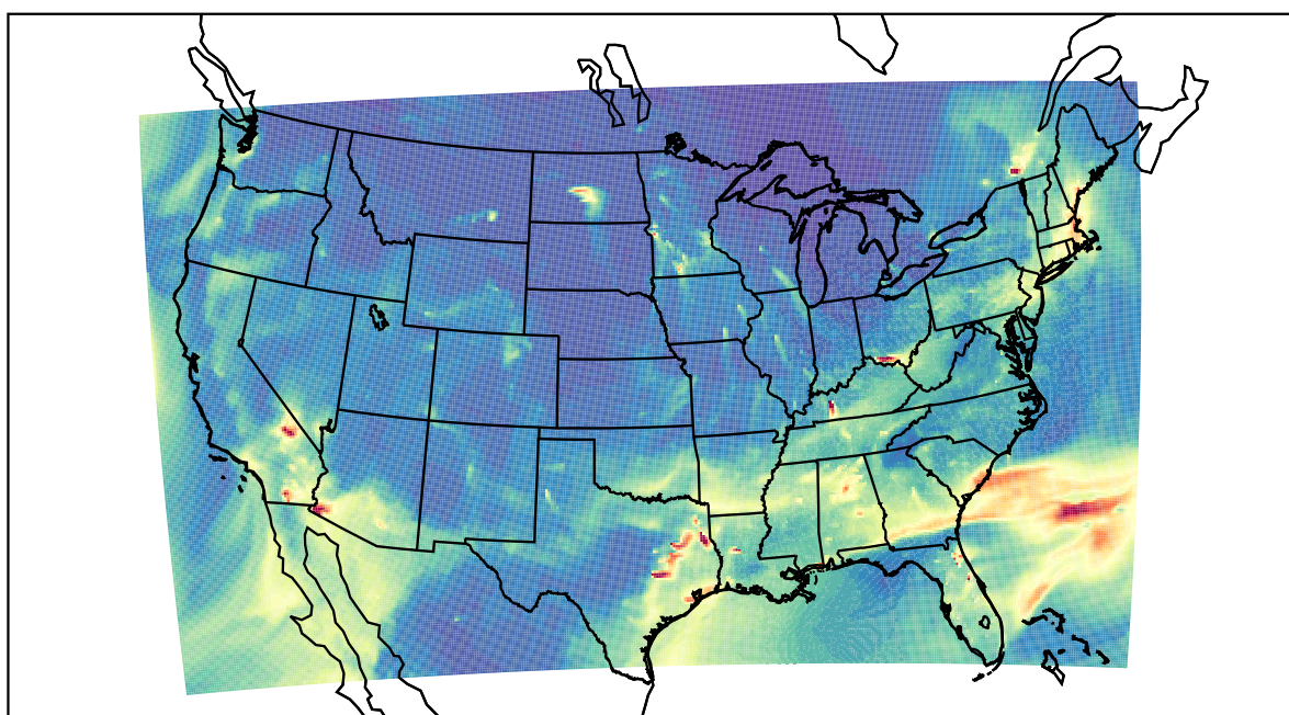
WRF 2021-01-22_12:00:00
