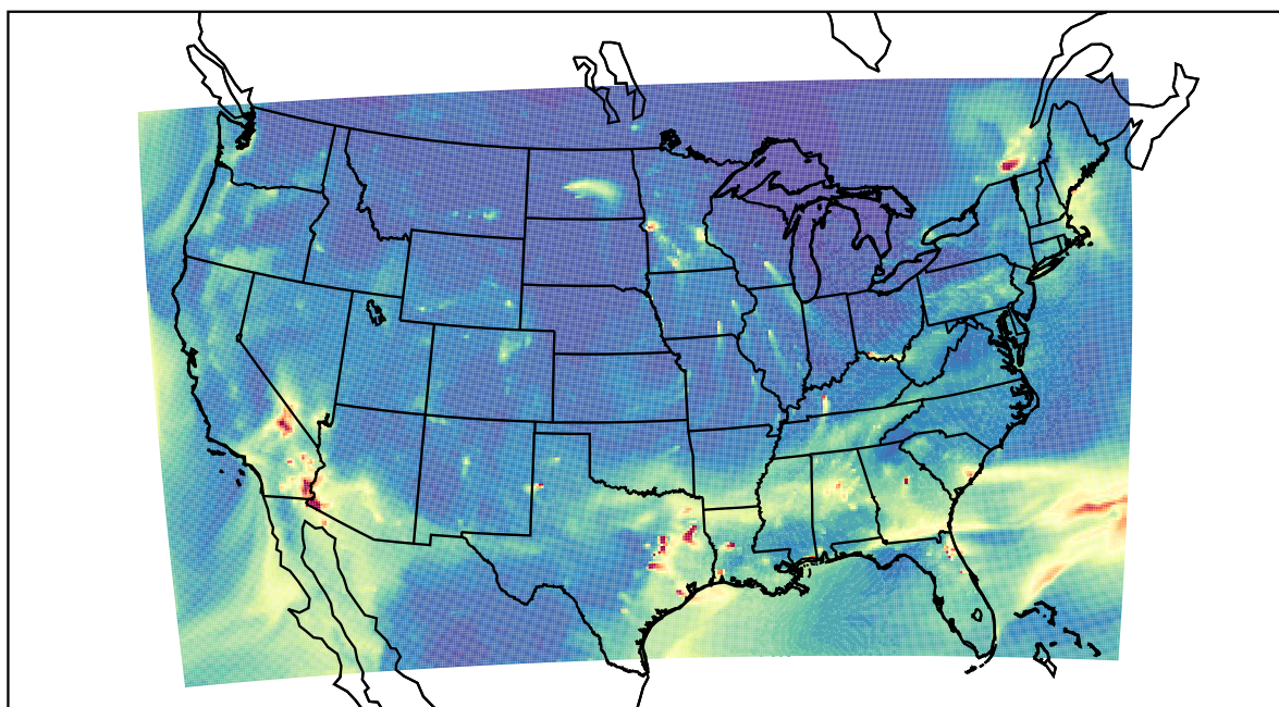
WRF 2021-01-22_16:00:00
