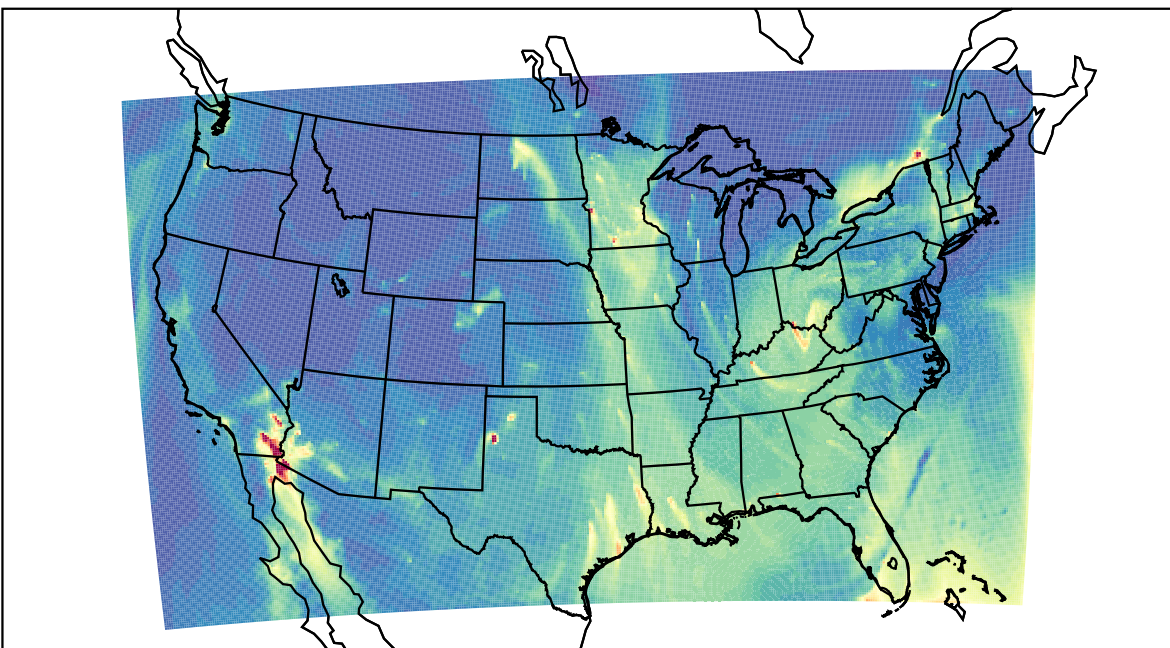
WRF 2021-02-01_11:00:00
