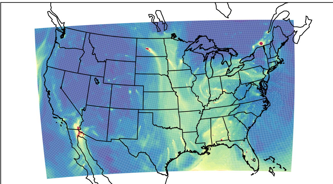
WRF 2021-01-31_18:00:00
