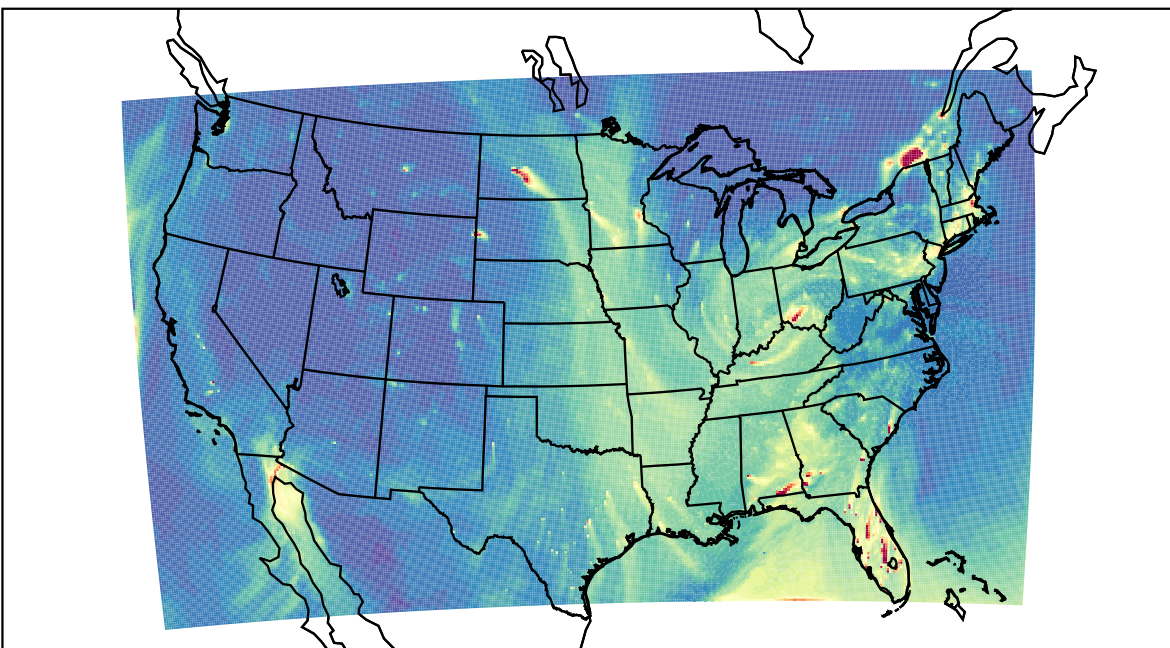
WRF 2021-01-31_23:00:00
