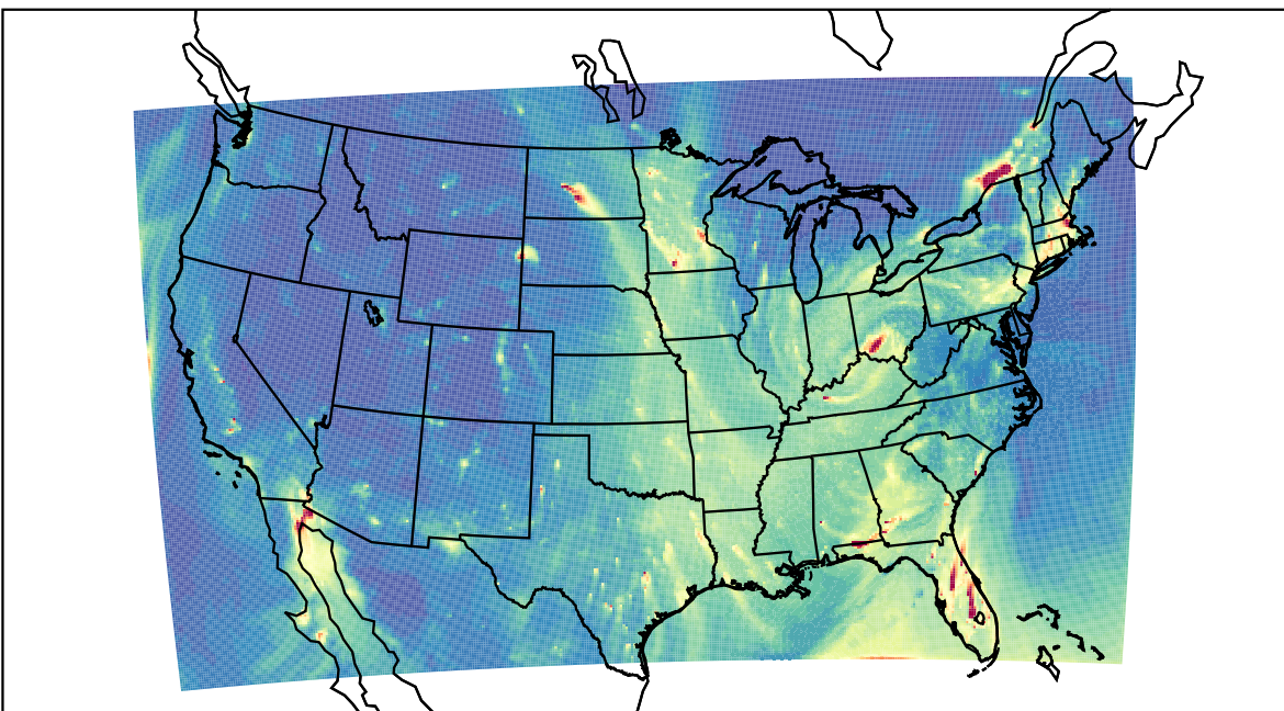
WRF 2021-02-01_01:00:00
