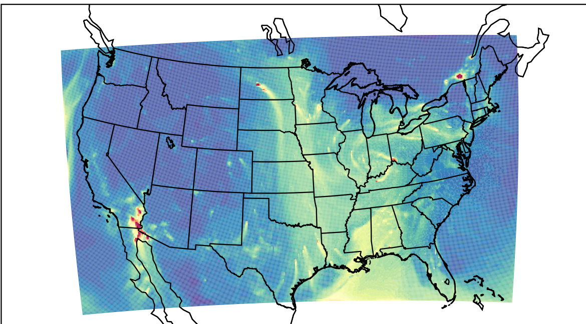
WRF 2021-01-31_16:00:00
