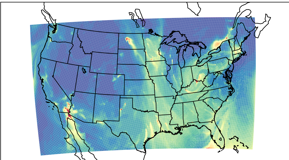
WRF 2021-02-01_08:00:00
