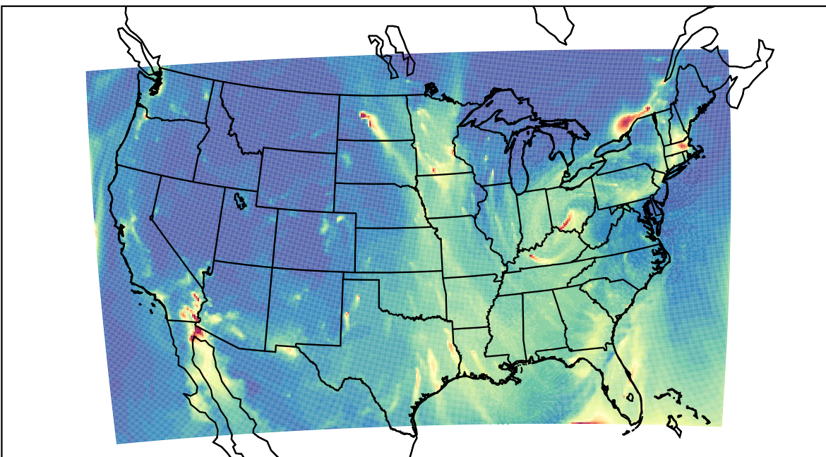
WRF 2021-02-01_06:00:00
