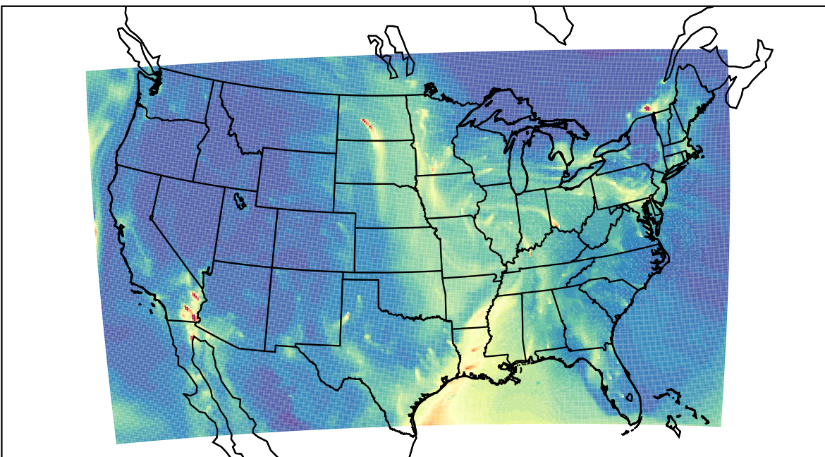
WRF 2021-01-31_10:00:00
