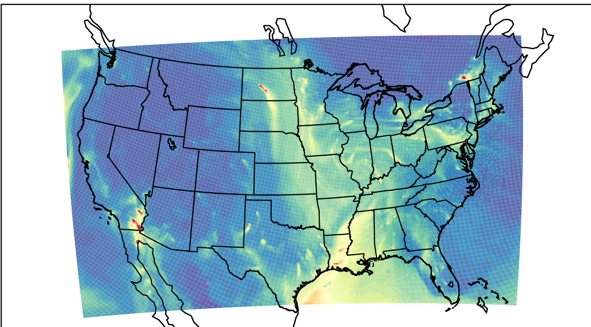
WRF 2021-01-31_11:00:00
