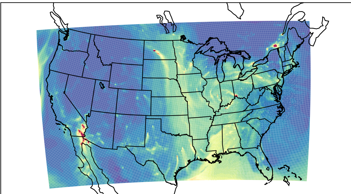
WRF 2021-01-31_15:00:00
