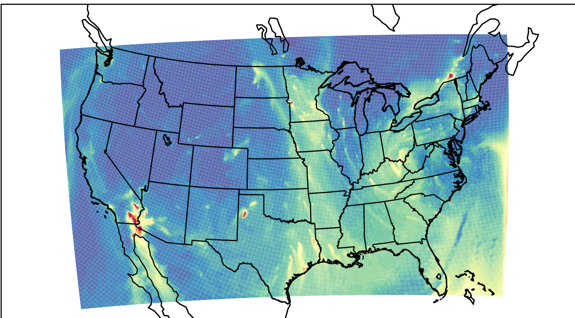
WRF 2021-02-01_13:00:00
