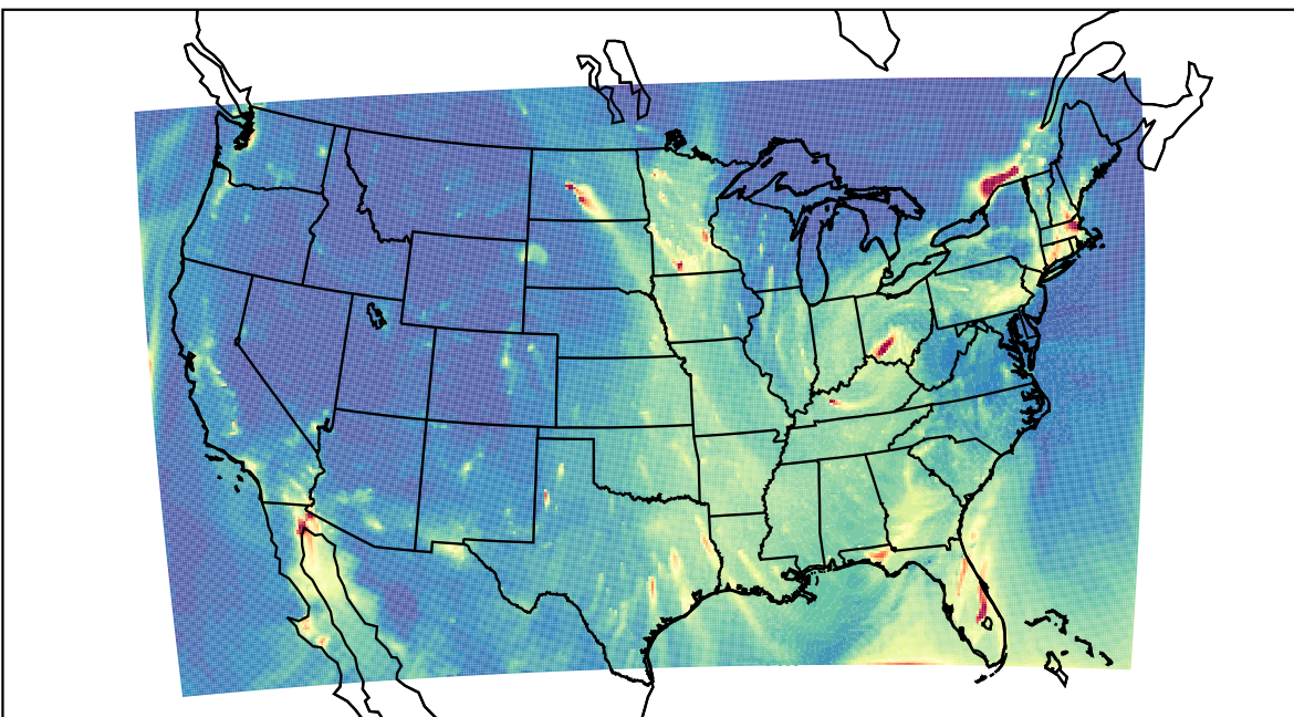
WRF 2021-02-01_03:00:00
