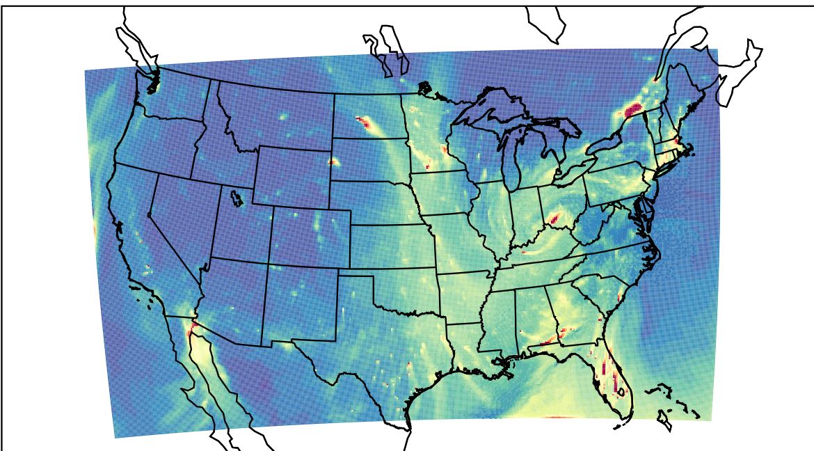
WRF 2021-02-01_00:00:00
