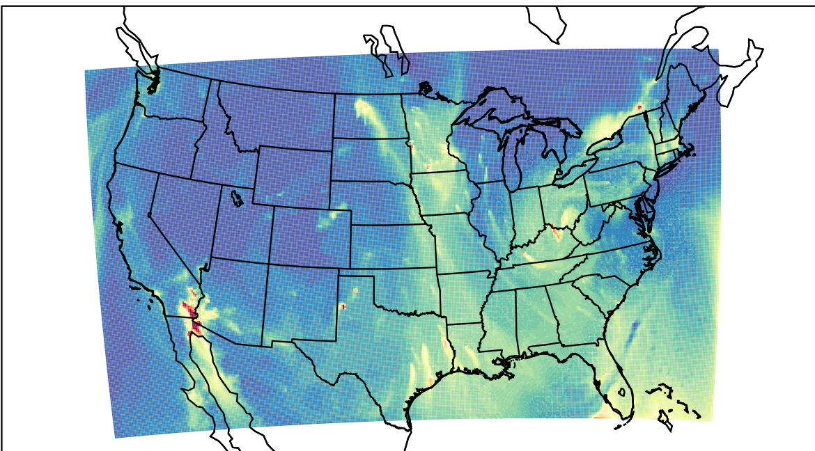
WRF 2021-02-01_10:00:00
