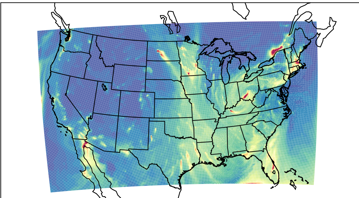
WRF 2021-02-01_04:00:00
