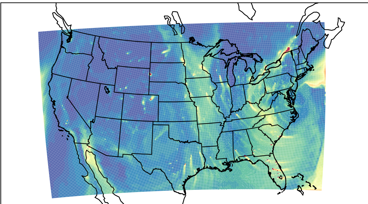
WRF 2021-02-01_23:00:00
