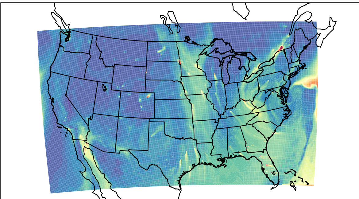
WRF 2021-02-01_20:00:00
