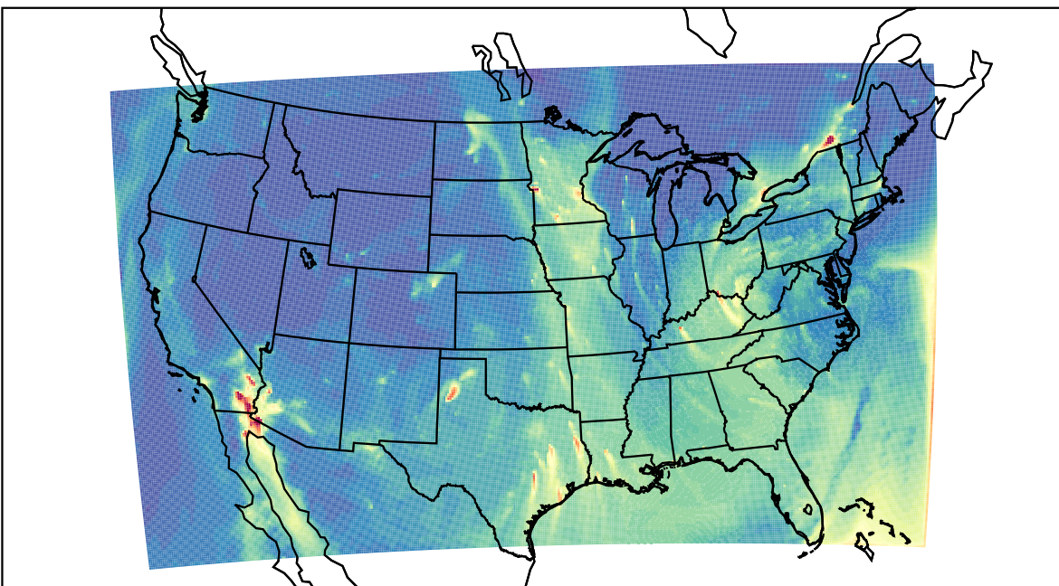
WRF 2021-02-01_14:00:00
