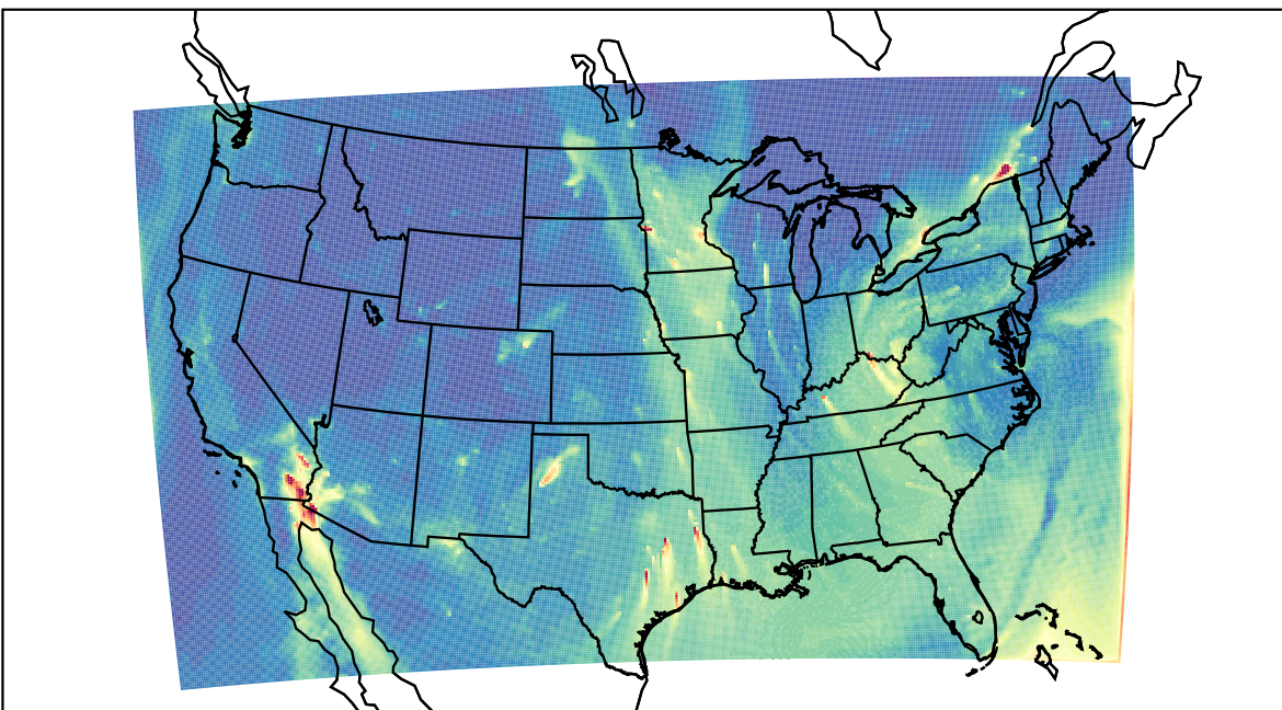
WRF 2021-02-01_15:00:00
