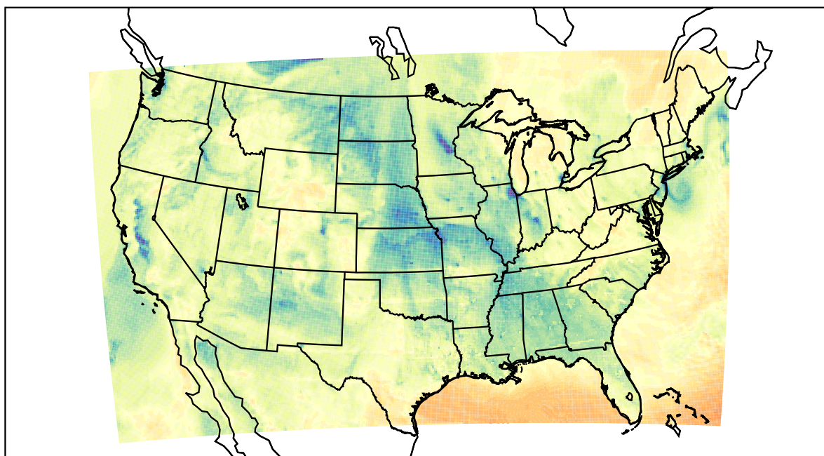
WRF (2021-02-02_23:00:00)
