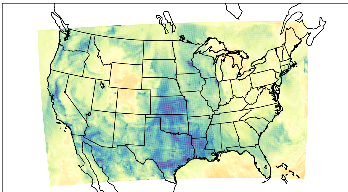
WRF (2021-02-02_14:00:00)
