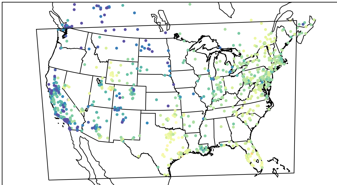
AirNOW (2021-02-03_18:00:00)
