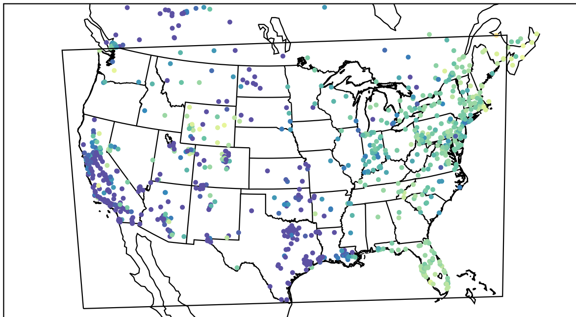
AirNOW (2021-02-02_14:00:00)
