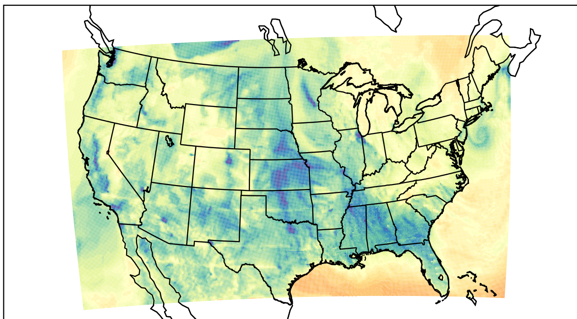
WRF (2021-02-03_03:00:00)
