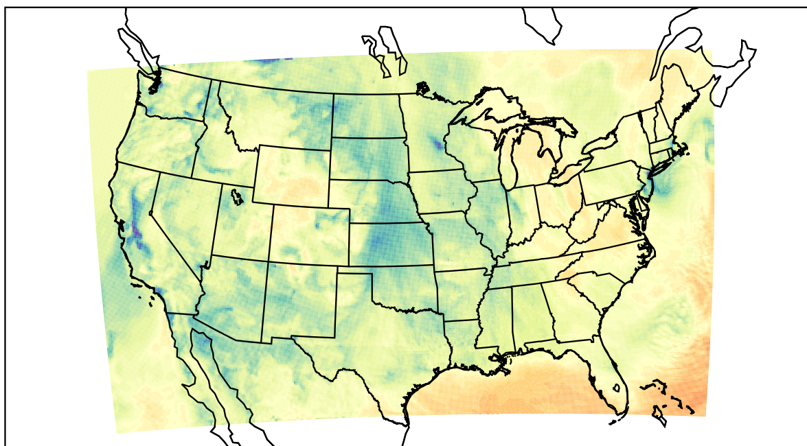
WRF (2021-02-02_19:00:00)
