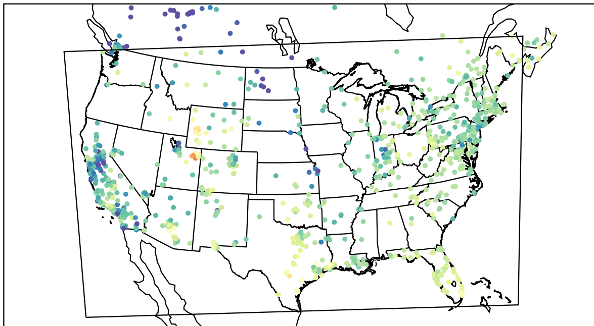
AirNOW (2021-02-02_20:00:00)
