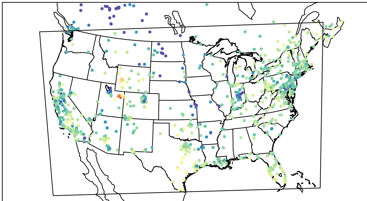
AirNOW (2021-02-02_23:00:00)
