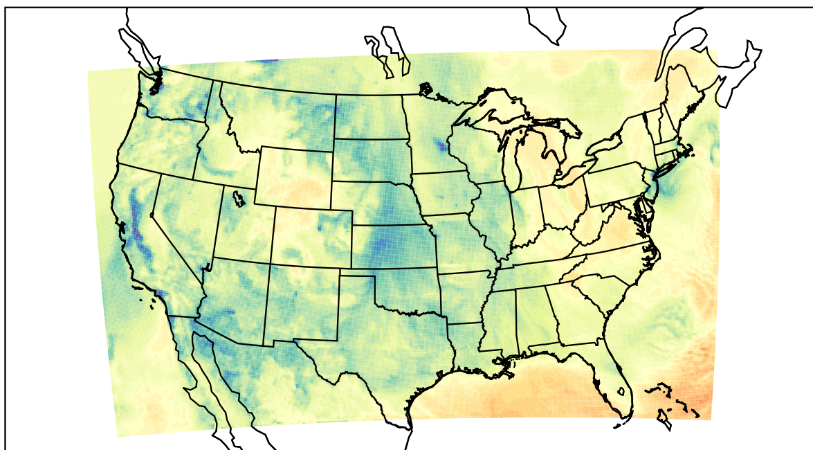
WRF (2021-02-02_18:00:00)
