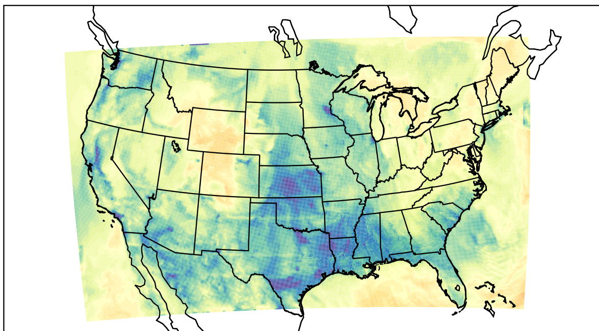
WRF (2021-02-02_13:00:00)
