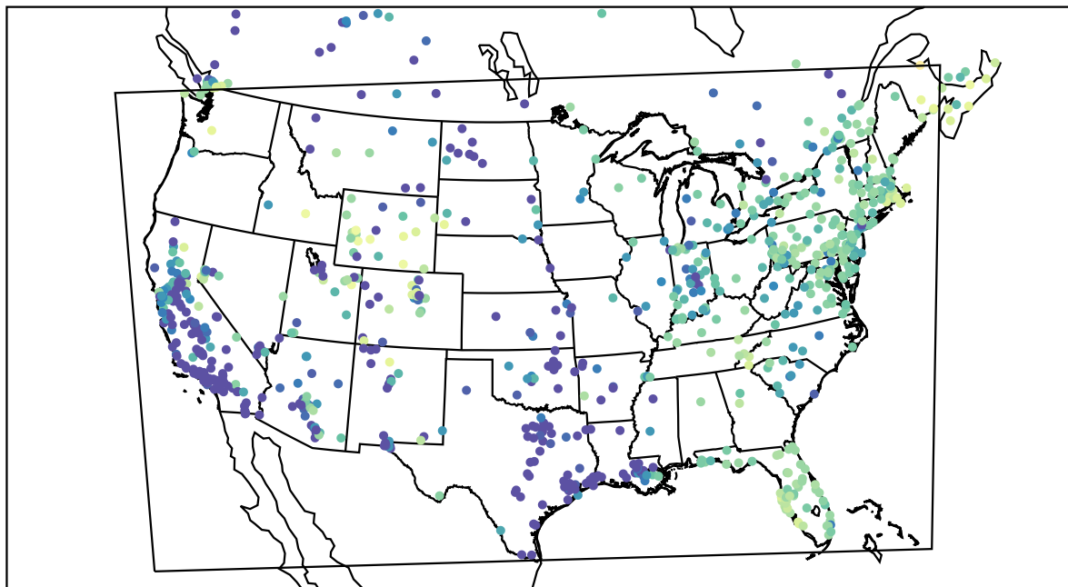
AirNOW (2021-02-02_10:00:00)
