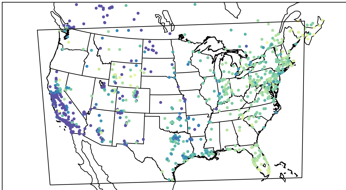
AirNOW (2021-02-02_16:00:00)
