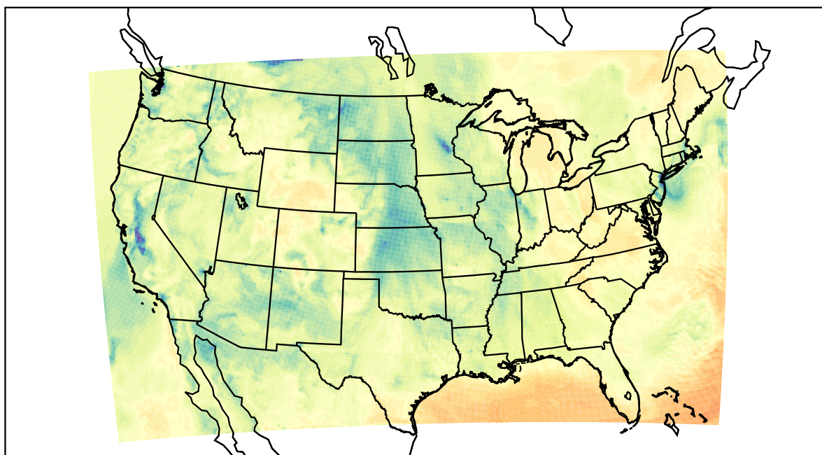
WRF (2021-02-02_20:00:00)
