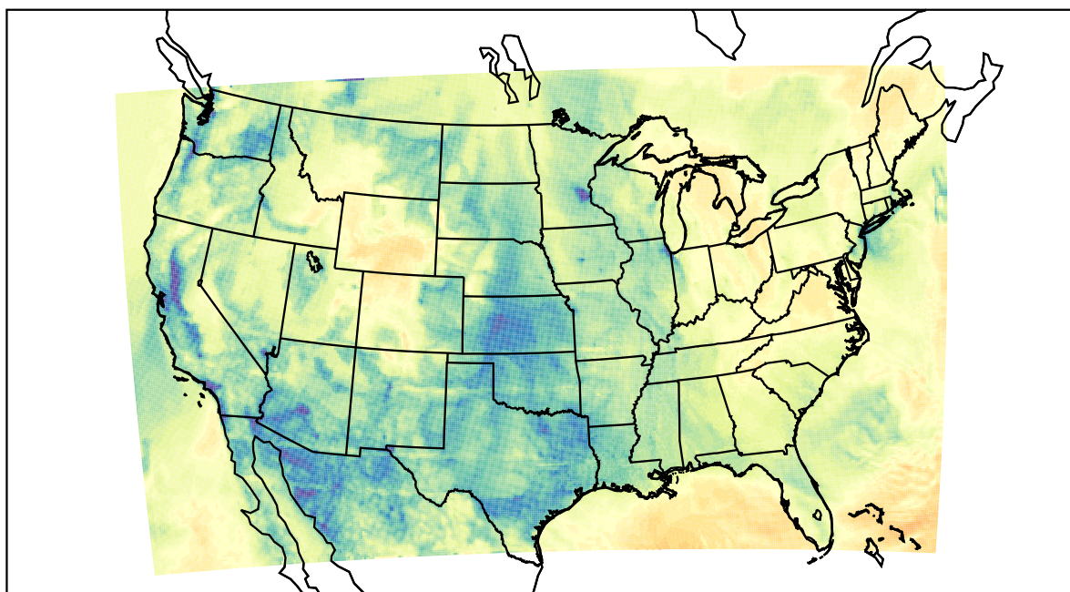
WRF (2021-02-02_16:00:00)
