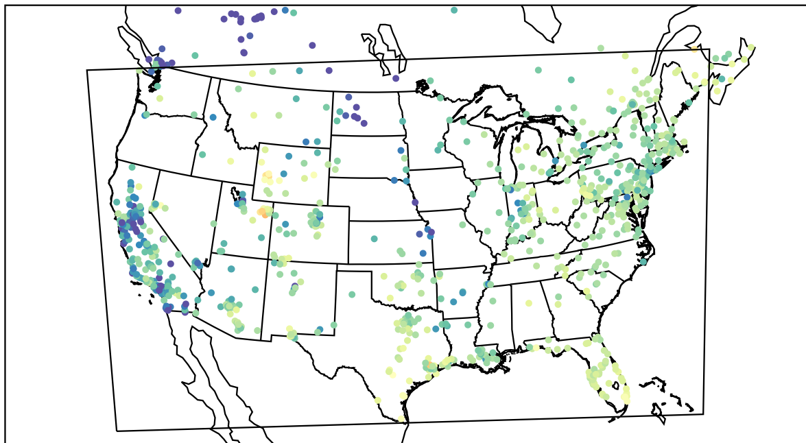
AirNOW (2021-02-02_19:00:00)
