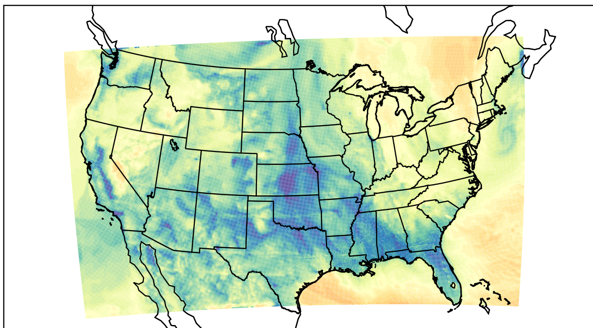
WRF (2021-02-03_10:00:00)
