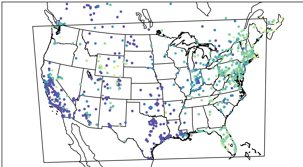
AirNOW (2021-02-02_13:00:00)
