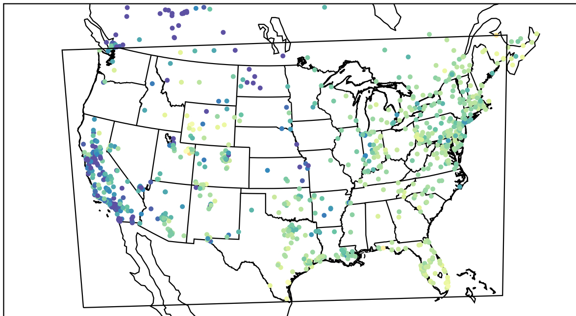
AirNOW (2021-02-02_18:00:00)
