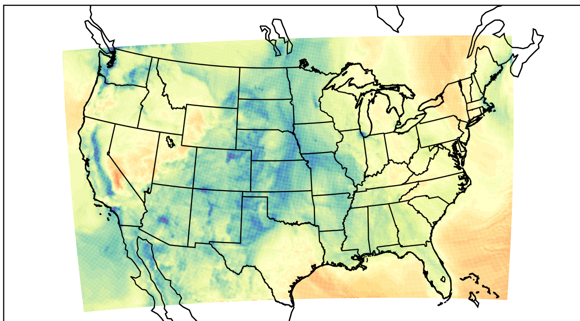
WRF (2021-02-03_18:00:00)
