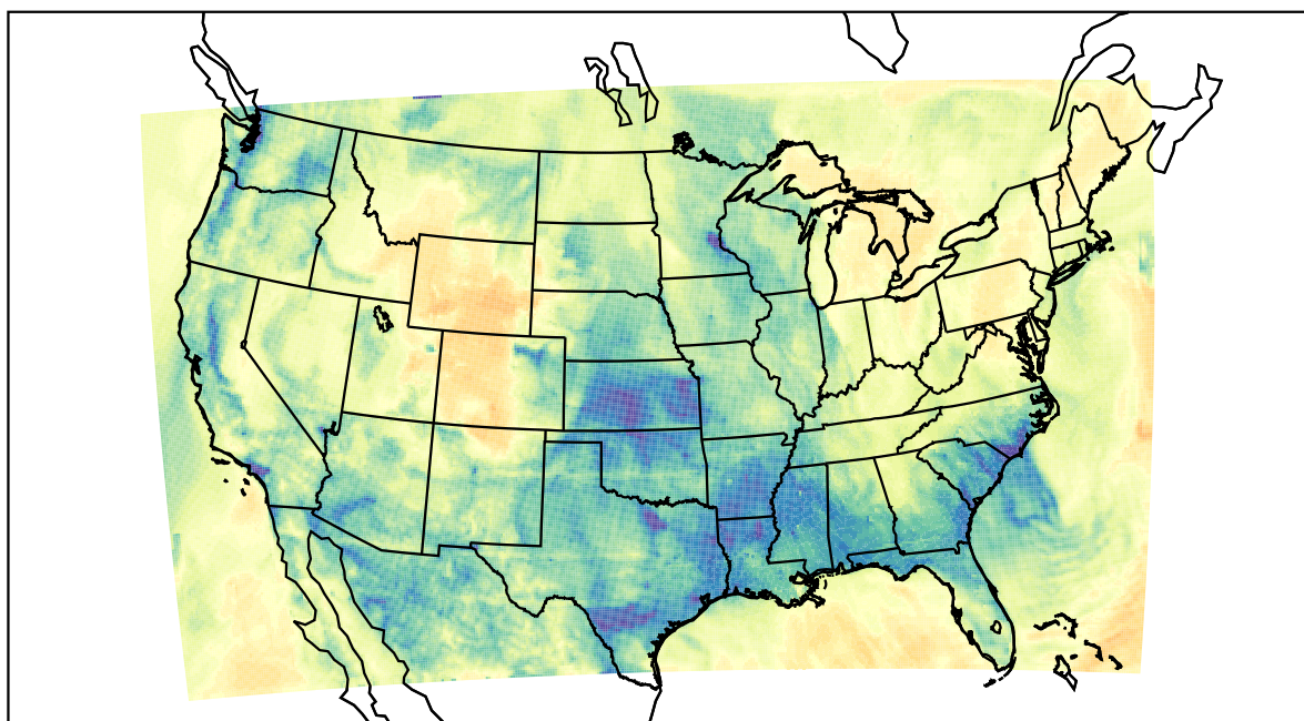
WRF (2021-02-02_10:00:00)
