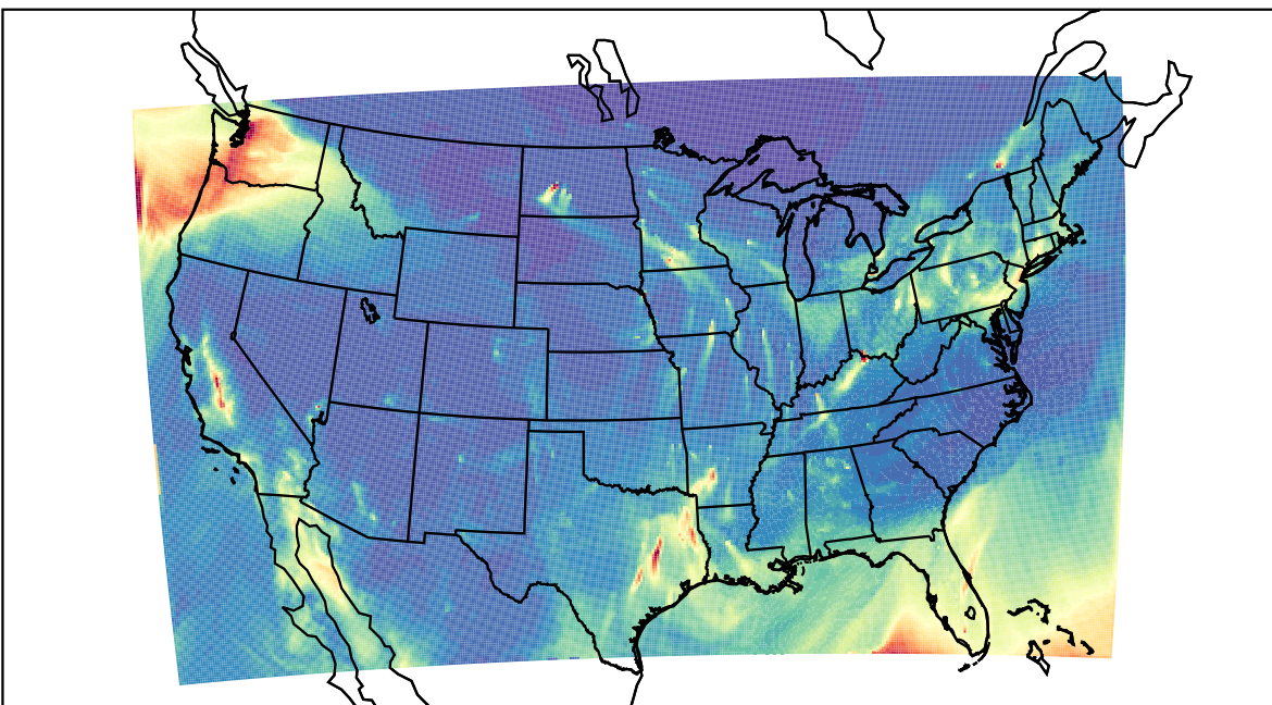
WRF 2021-02-07_08:00:00
