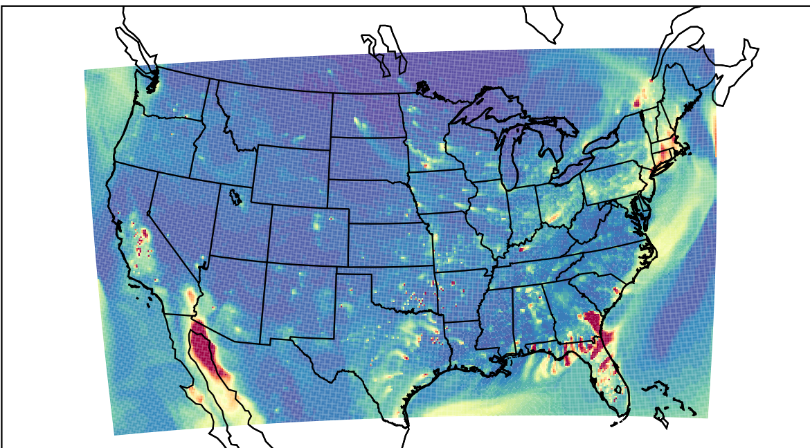
WRF 2021-02-06_01:00:00
