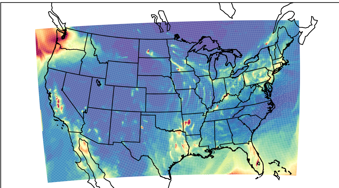
WRF 2021-02-07_04:00:00
