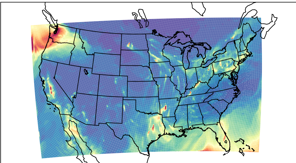
WRF 2021-02-07_06:00:00
