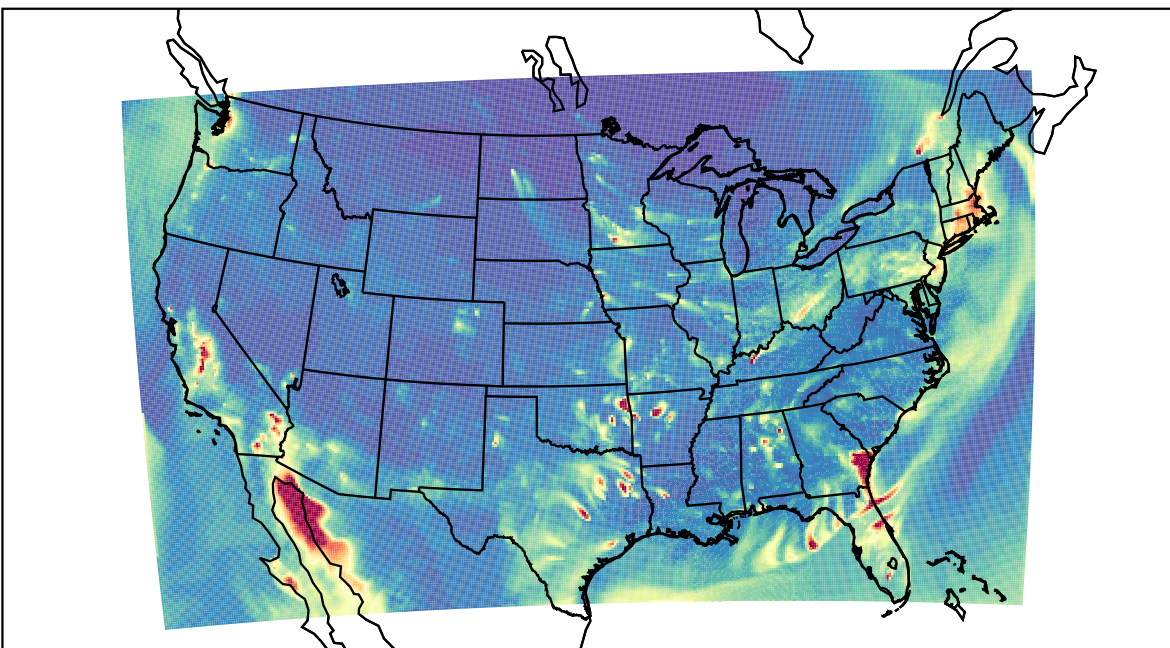
WRF 2021-02-06_04:00:00
