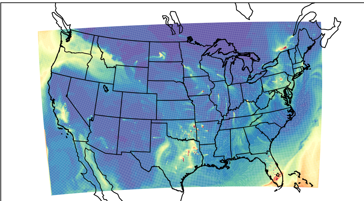
WRF 2021-02-07_20:00:00
