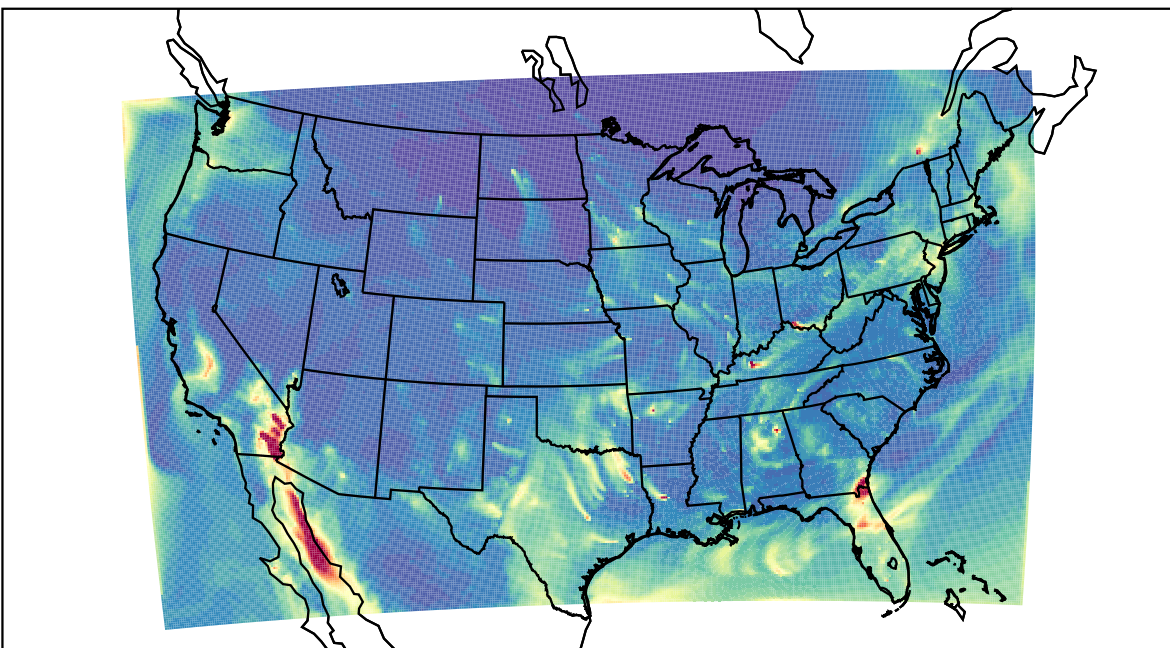
WRF 2021-02-06_10:00:00
