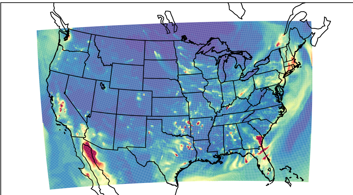
WRF 2021-02-06_03:00:00
