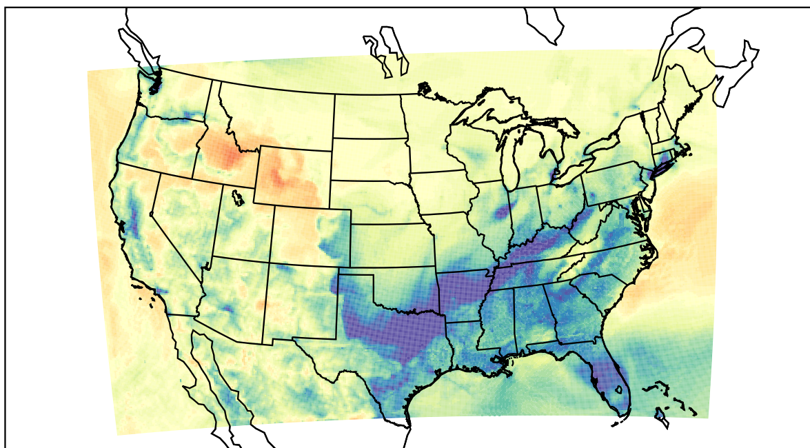
WRF (2021-02-09_10:00:00)
