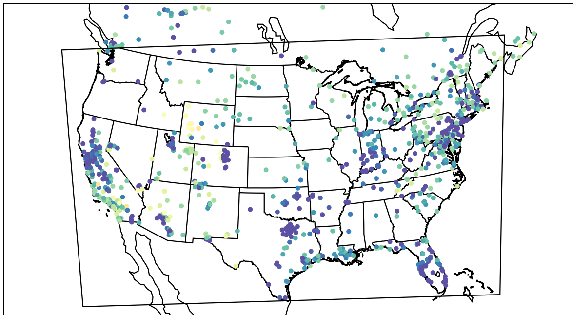
AirNOW (2021-02-09_03:00:00)
