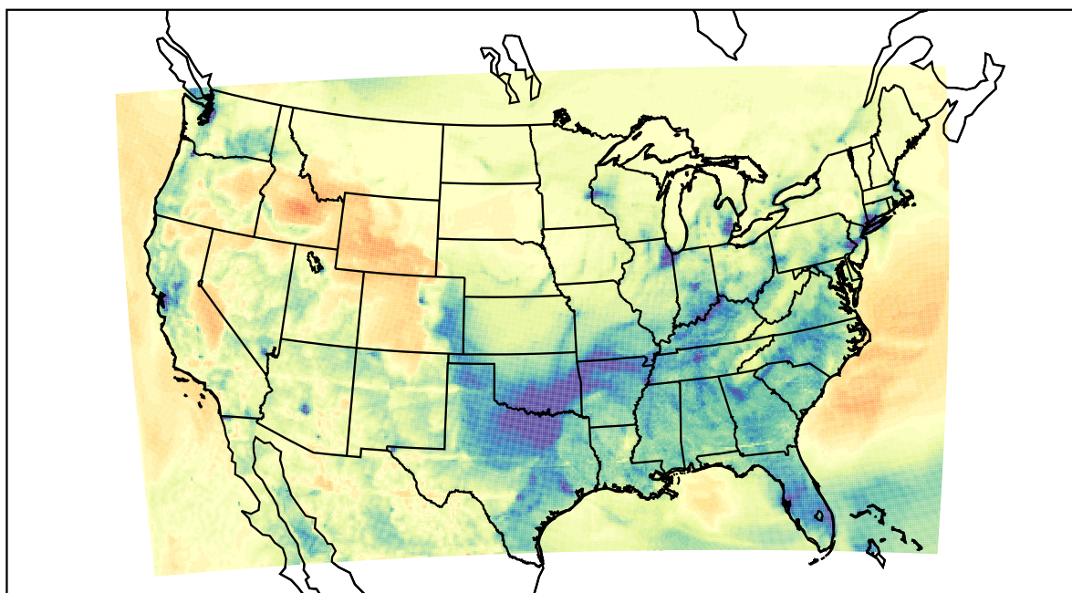
WRF (2021-02-09_03:00:00)
