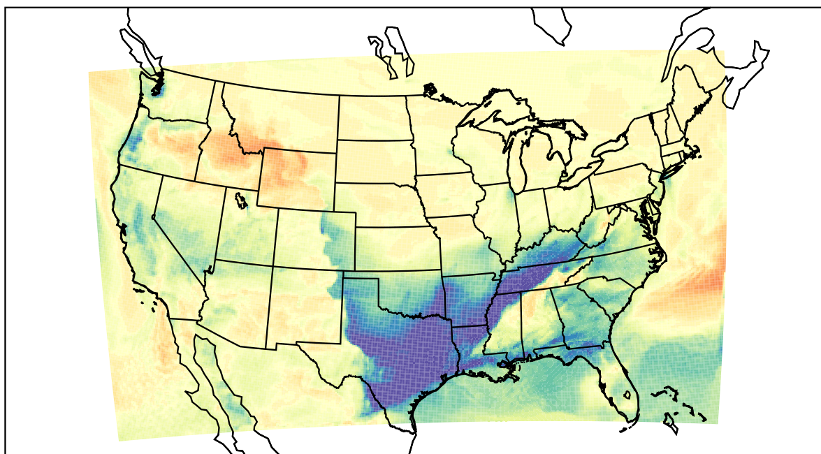
WRF (2021-02-10_20:00:00)
