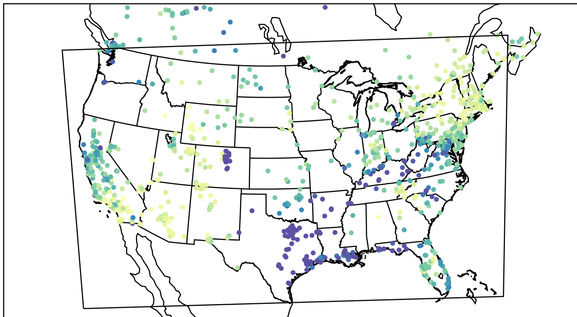
AirNOW (2021-02-10_20:00:00)
