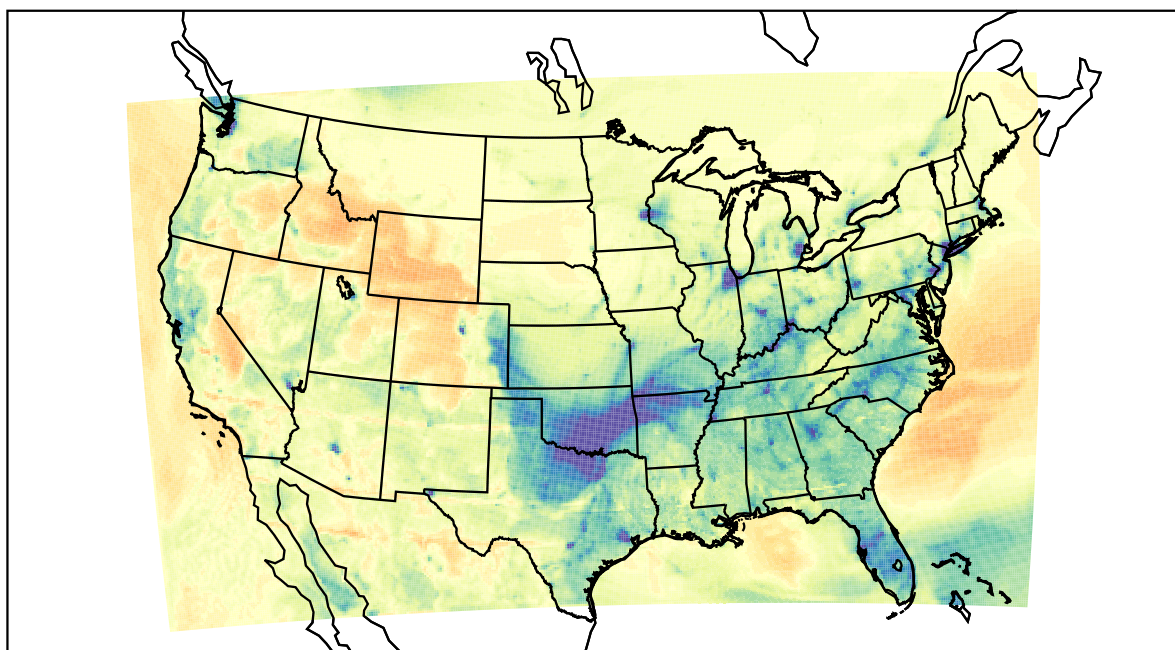
WRF (2021-02-09_01:00:00)
