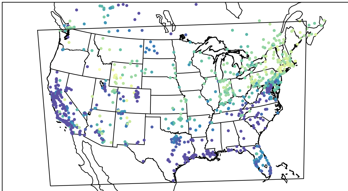
AirNOW (2021-02-11_16:00:00)
