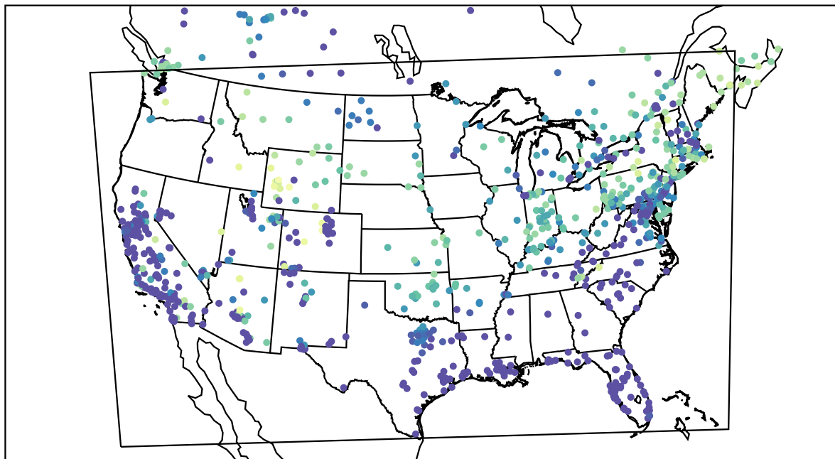
AirNOW (2021-02-11_13:00:00)
