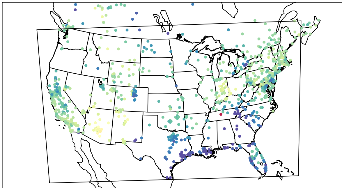
AirNOW (2021-02-12_20:00:00)
