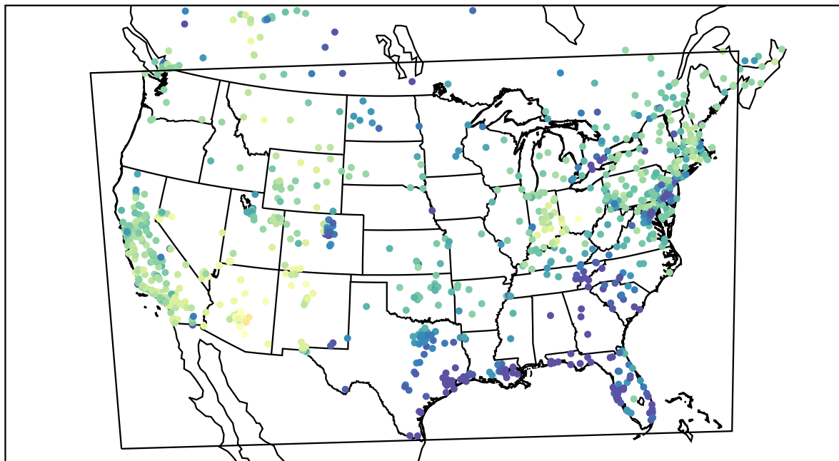
AirNOW (2021-02-12_23:00:00)
