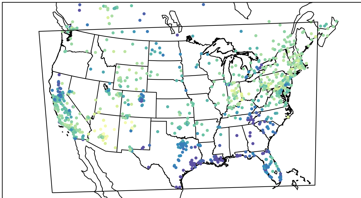
AirNOW (2021-02-12_18:00:00)
