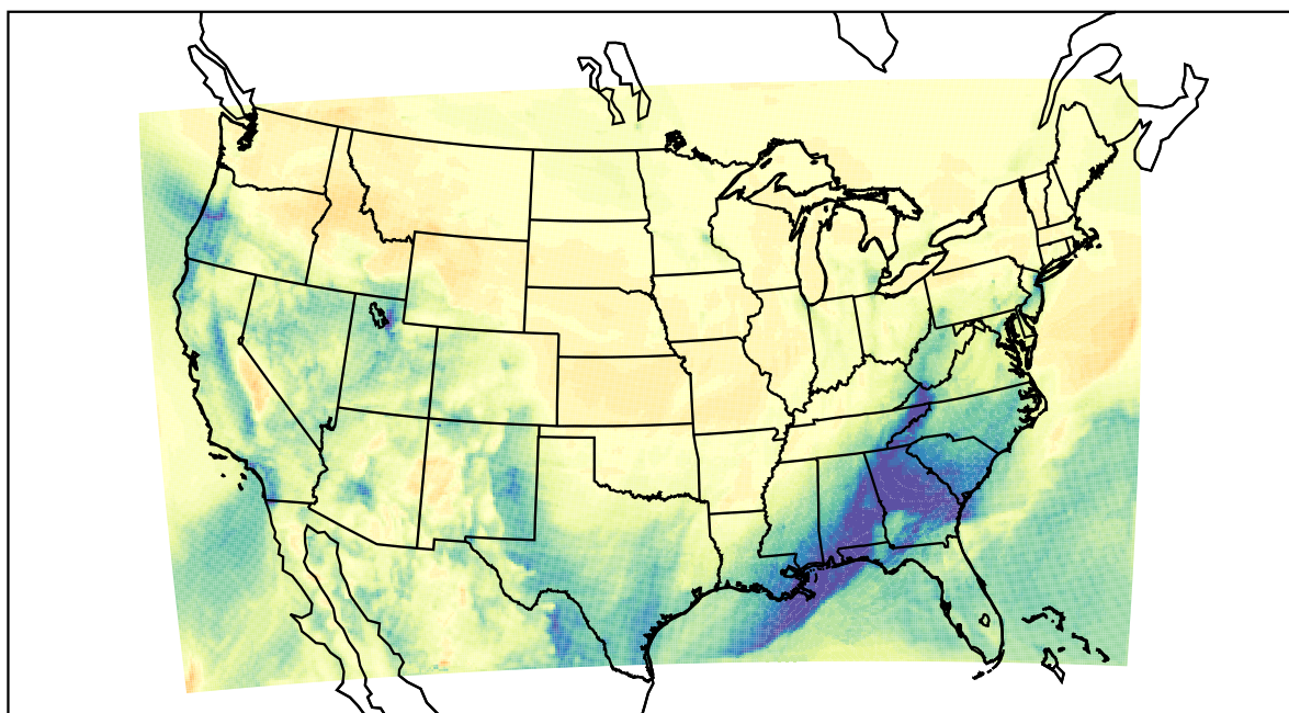
WRF (2021-02-12_18:00:00)
