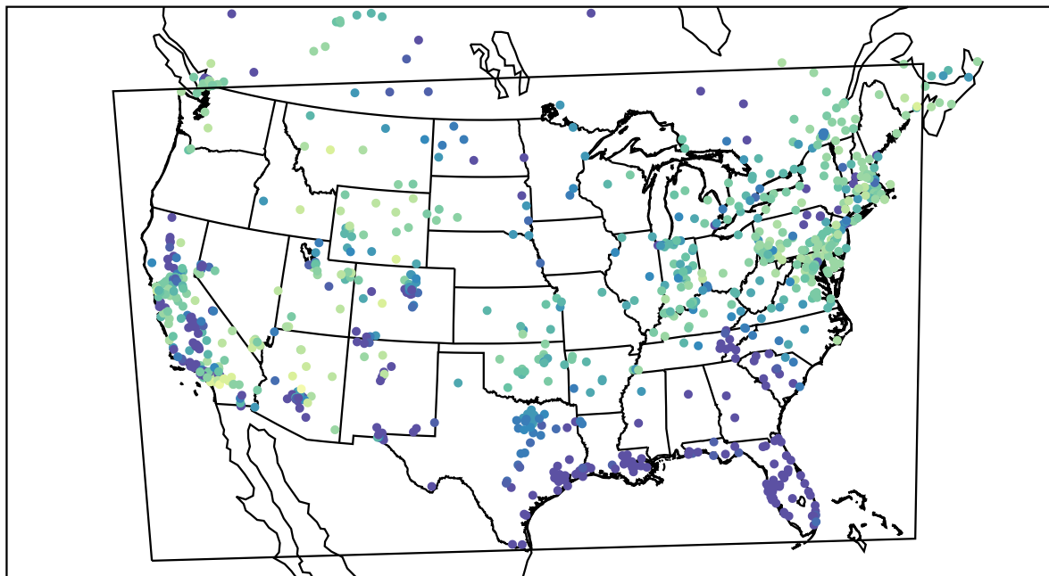
AirNOW (2021-02-12_10:00:00)
