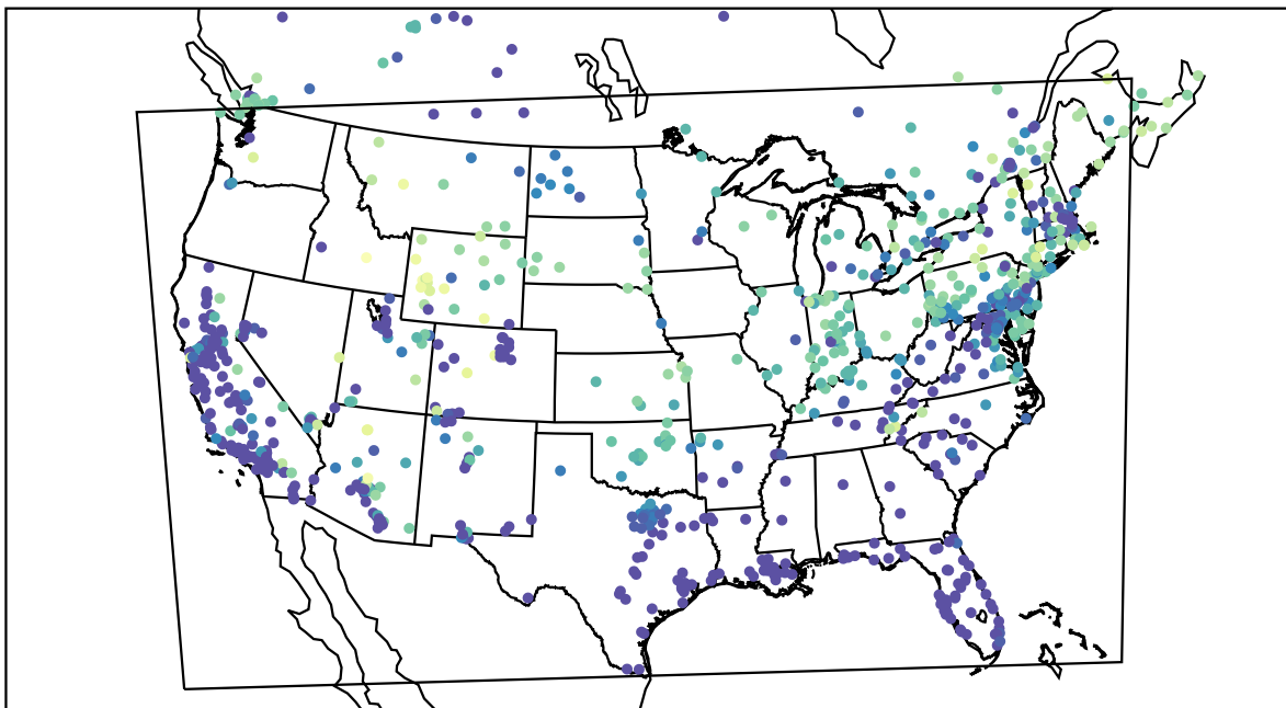
AirNOW (2021-02-11_10:00:00)
