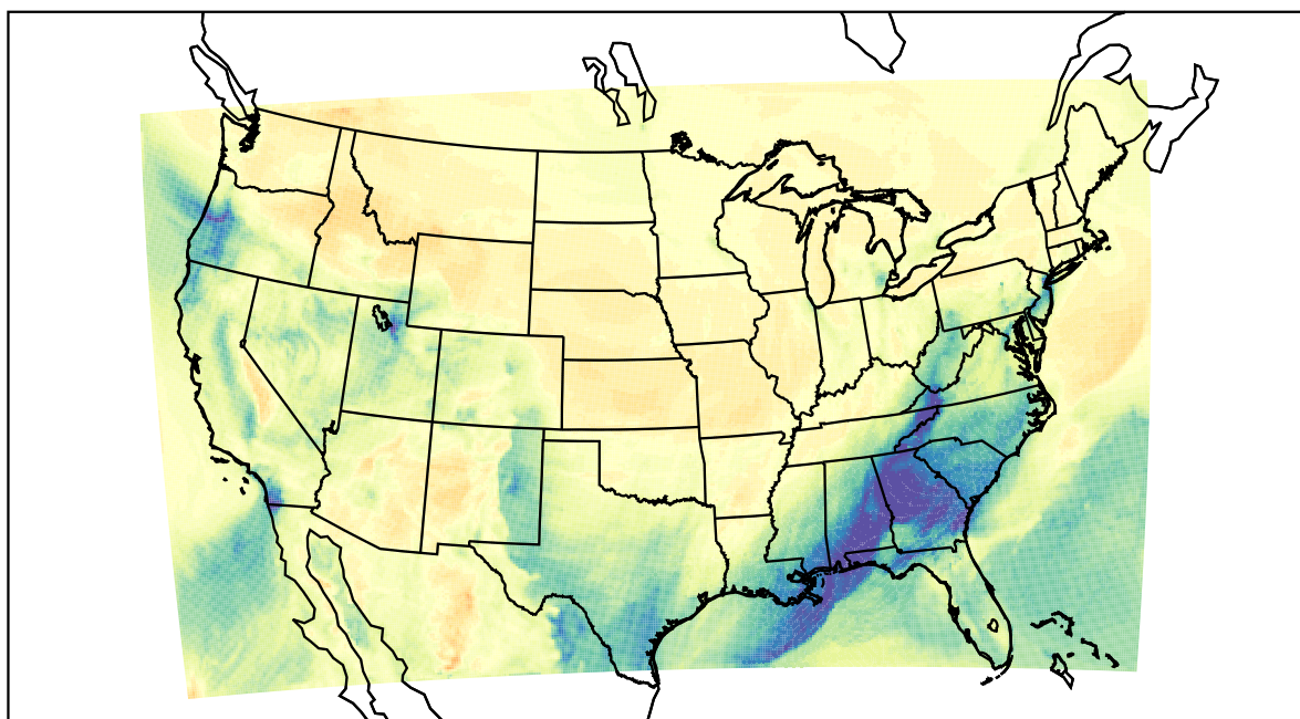
WRF (2021-02-12_20:00:00)
