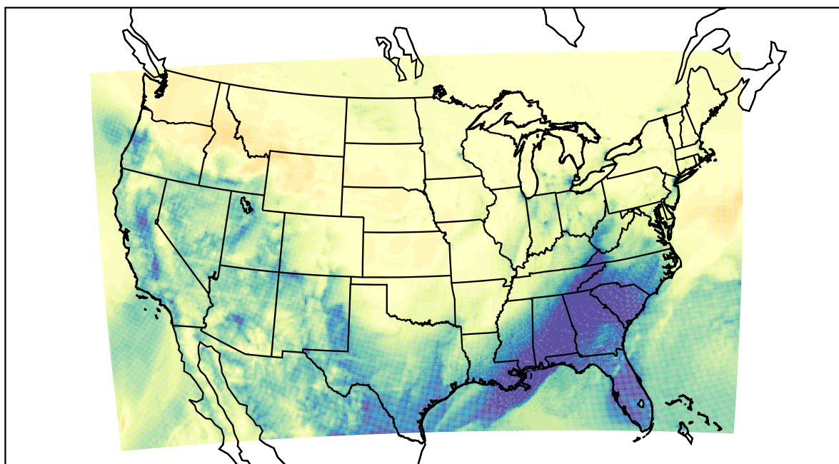
WRF (2021-02-12_13:00:00)
