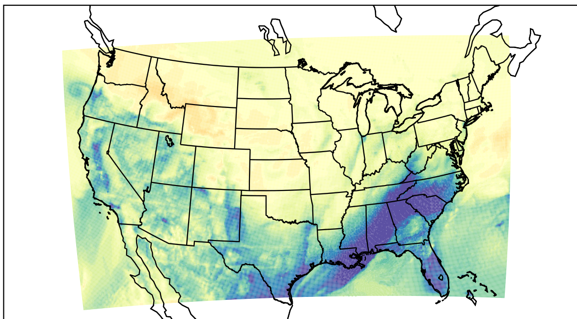
WRF (2021-02-12_10:00:00)
