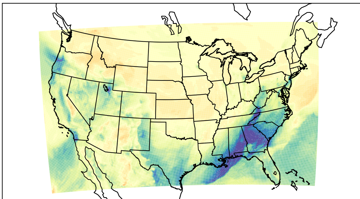
WRF (2021-02-12_19:00:00)
