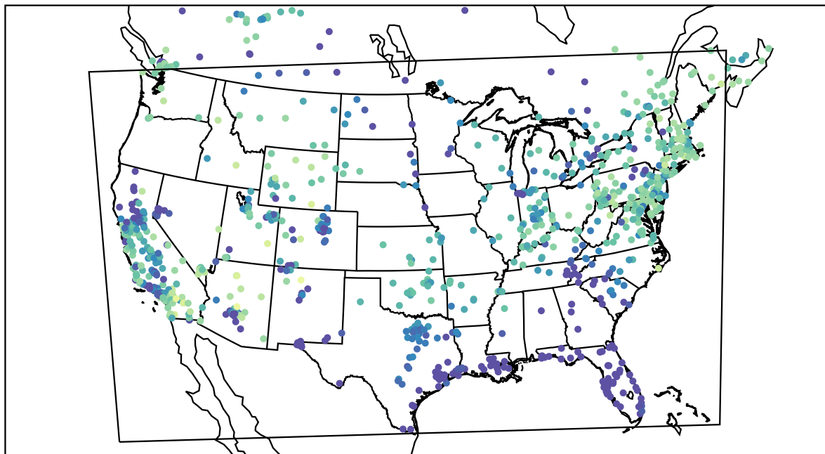
AirNOW (2021-02-12_13:00:00)
