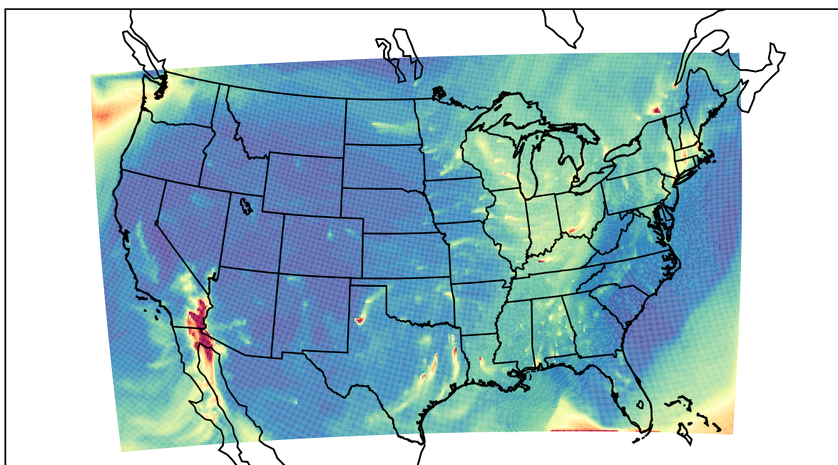
WRF 2021-02-22_14:00:00
