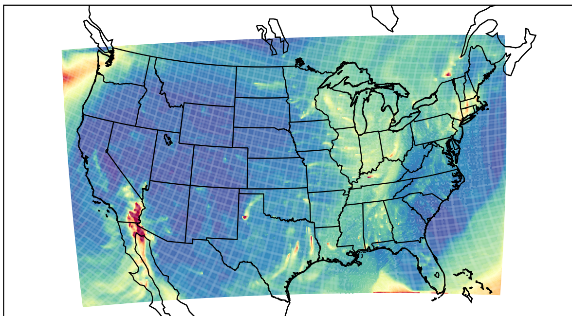
WRF 2021-02-22_13:00:00
