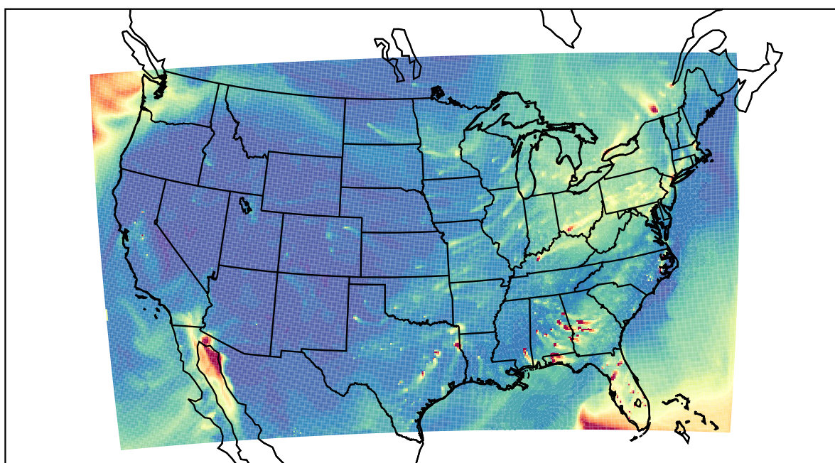
WRF 2021-02-22_23:00:00
