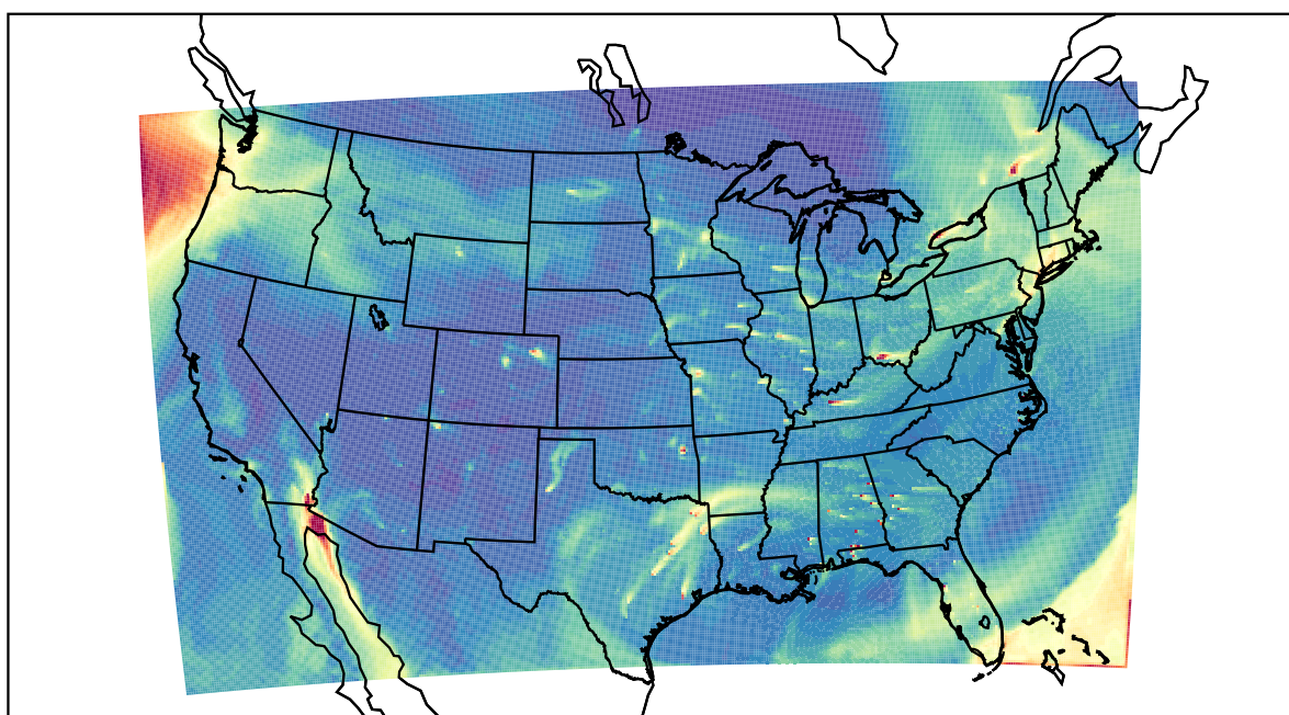
WRF 2021-02-23_18:00:00
