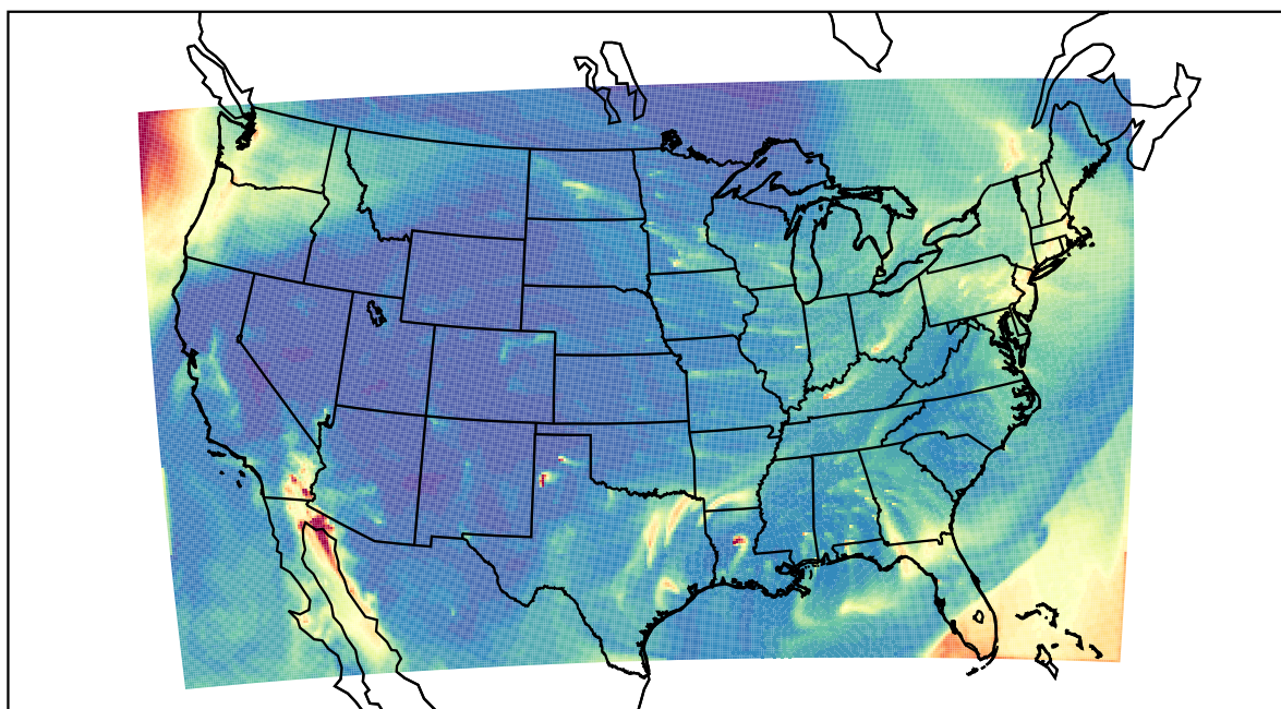
WRF 2021-02-23_10:00:00
