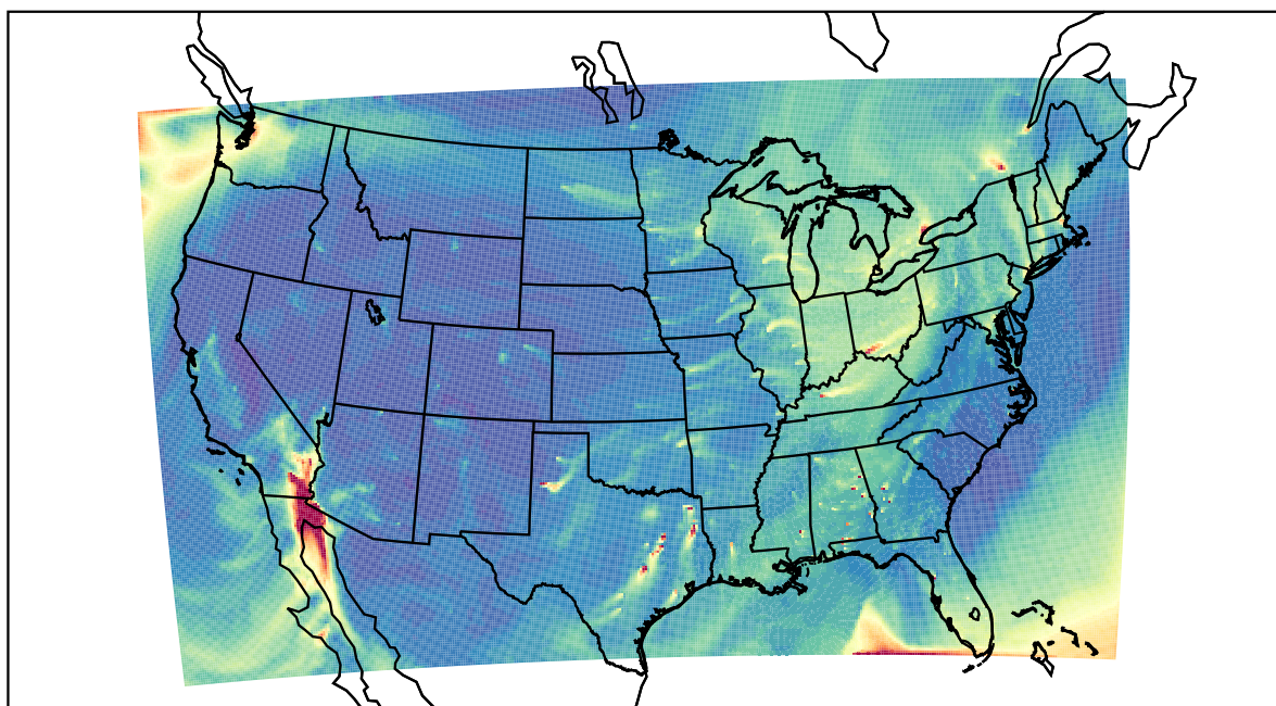
WRF 2021-02-22_17:00:00
