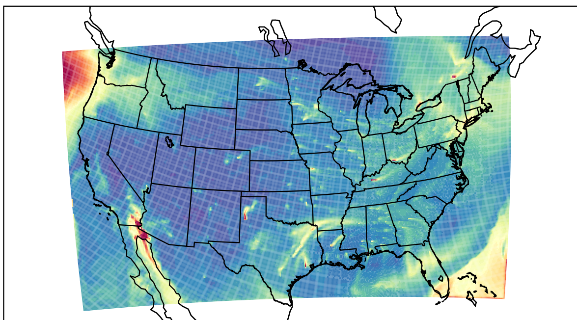
WRF 2021-02-23_15:00:00
