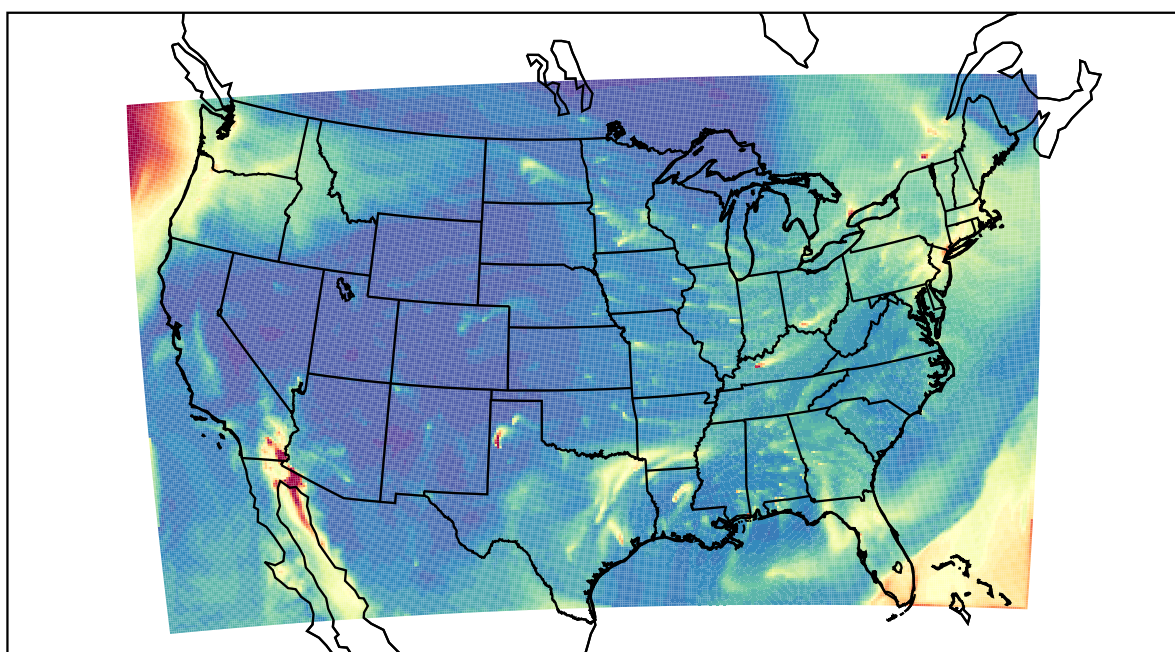
WRF 2021-02-23_13:00:00
