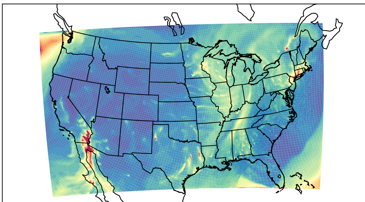
WRF 2021-02-22_10:00:00
