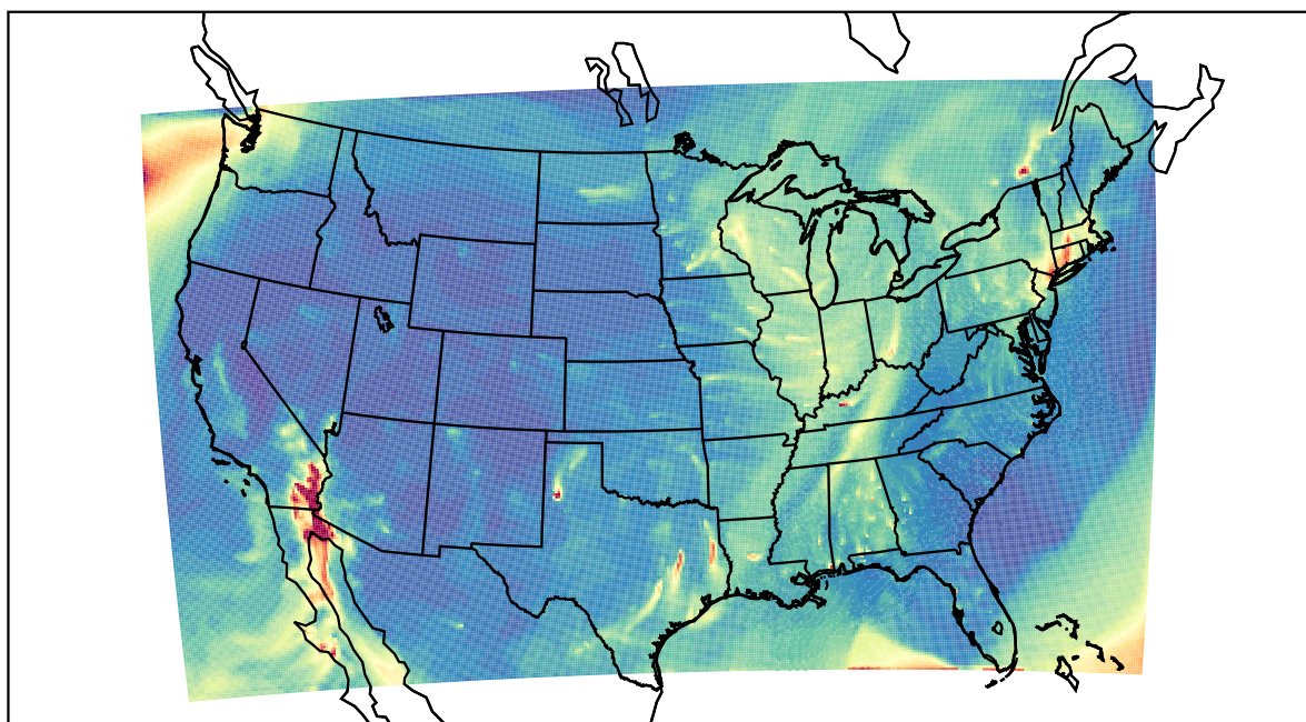
WRF 2021-02-22_11:00:00
