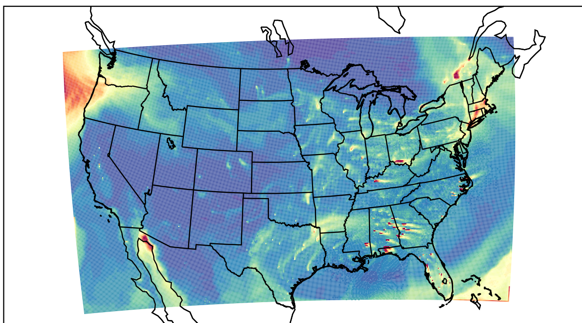
WRF 2021-02-23_23:00:00
