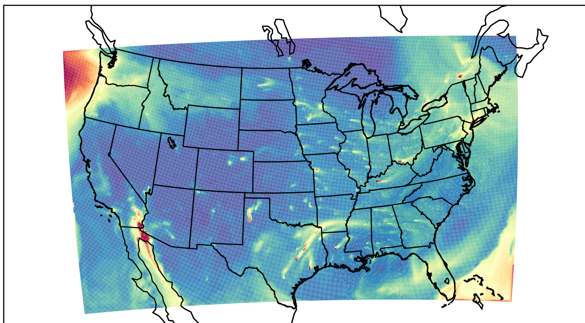
WRF 2021-02-23_16:00:00
