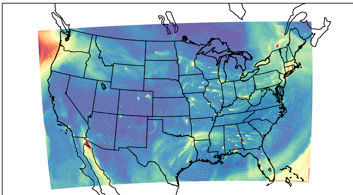
WRF 2021-02-23_20:00:00
