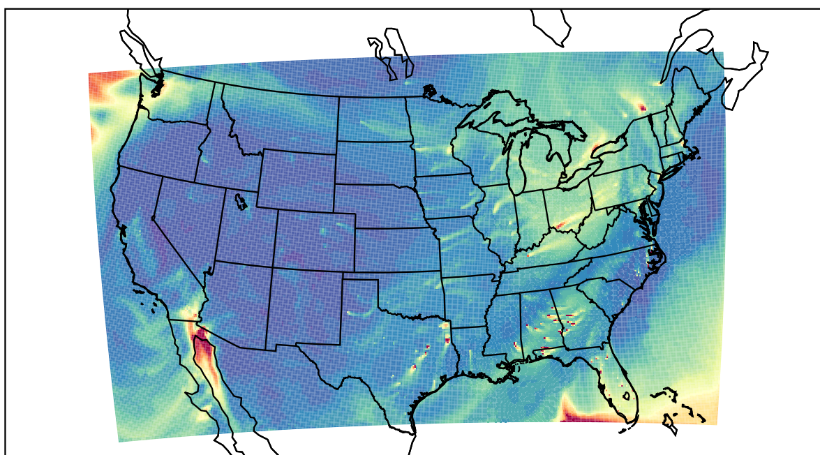
WRF 2021-02-22_20:00:00
