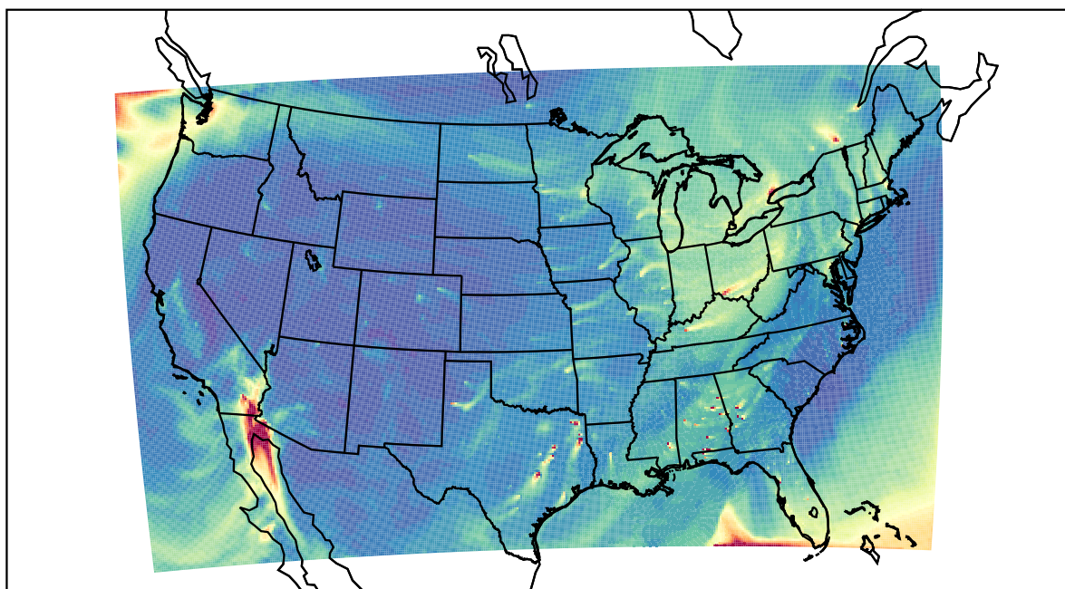
WRF 2021-02-22_18:00:00
