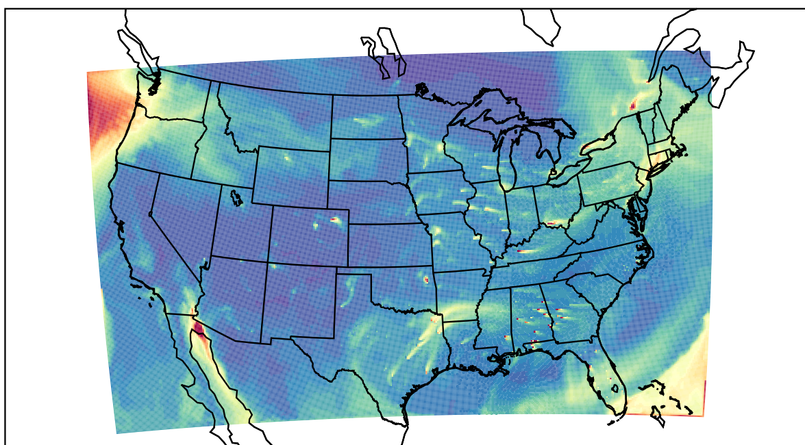
WRF 2021-02-23_19:00:00
