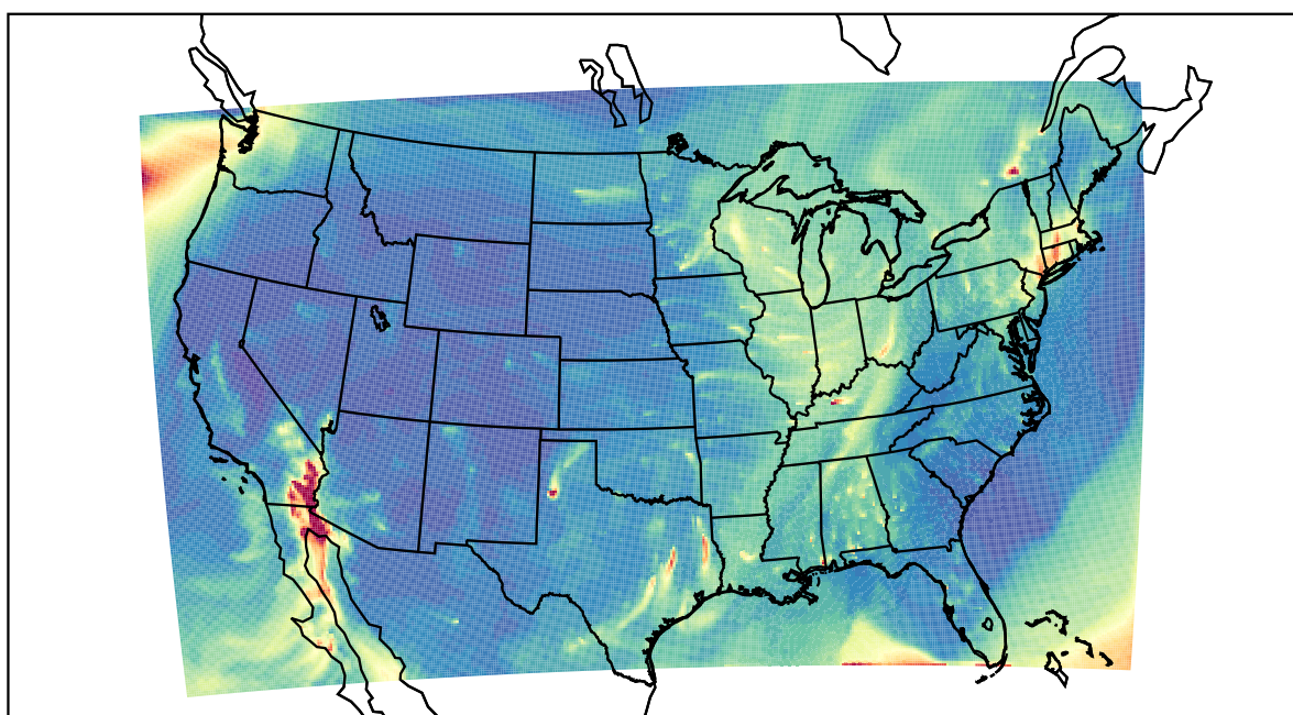
WRF 2021-02-22_12:00:00
