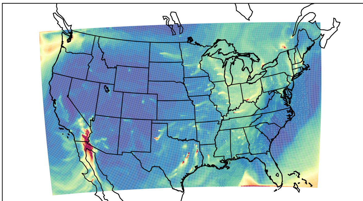
WRF 2021-02-22_16:00:00
