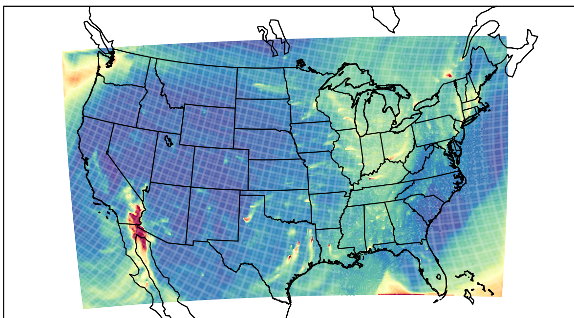
WRF 2021-02-22_15:00:00
