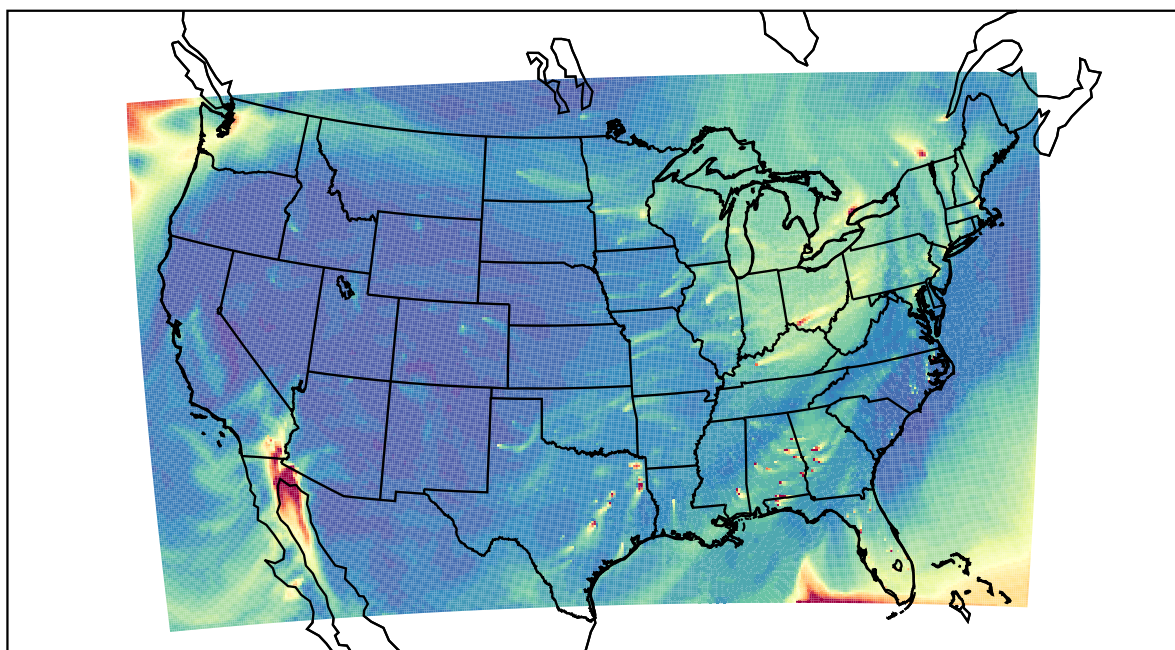
WRF 2021-02-22_19:00:00
