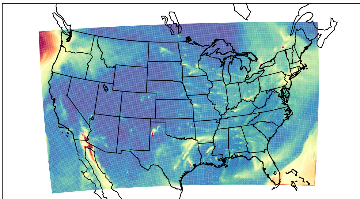
WRF 2021-02-23_14:00:00
